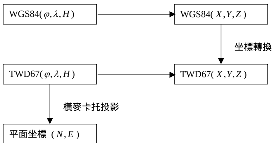
圖 2.4 坐標轉換及地圖投影流程
