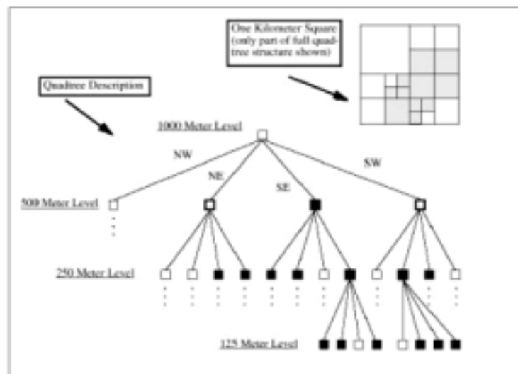
圖3.10 多層次精細度模型的四元樹
