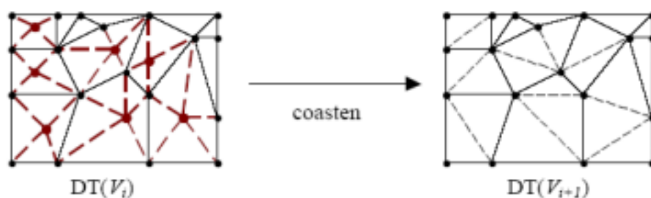
圖3.11 階層式的多層次精細度模型
