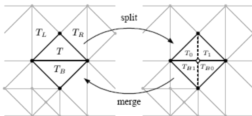
圖 3.17 三角二元樹結構之分割與合併操作
