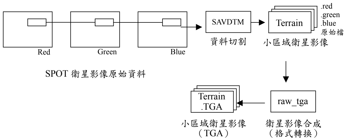
圖 3.4 數值影像切割與格式轉換作業流程
