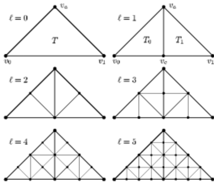
圖 3.13 ROAM 基本三角形結構(Level 0-5 三角二元樹)
