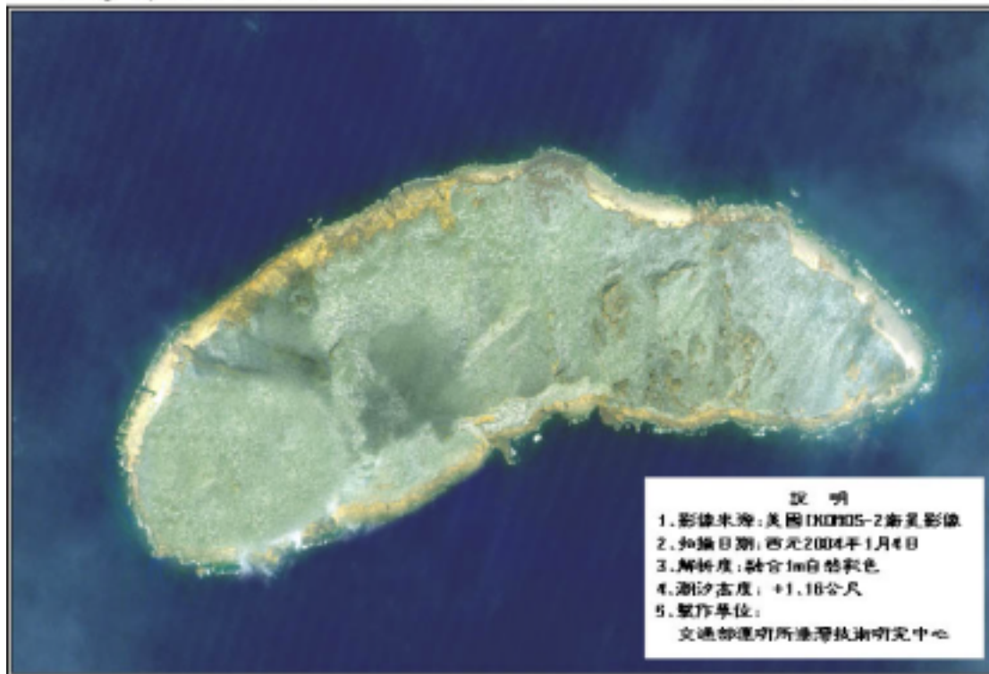
圖 5.5 釣魚台數值圖像
