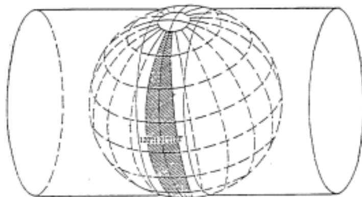
圖 2.5 橫麥卡脫投影
