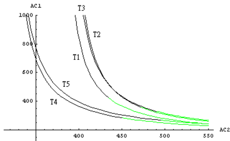
圖 8.8 曼谷港貨櫃經香港轉運之主航線的可行解
