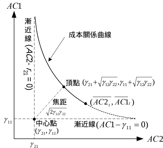
圖 6.2 任一型貨櫃船的柏拉圖最佳解
