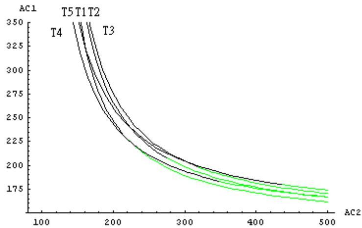
圖 8.7 曼谷港貨櫃經高雄港轉運之接駁航線的可行解
