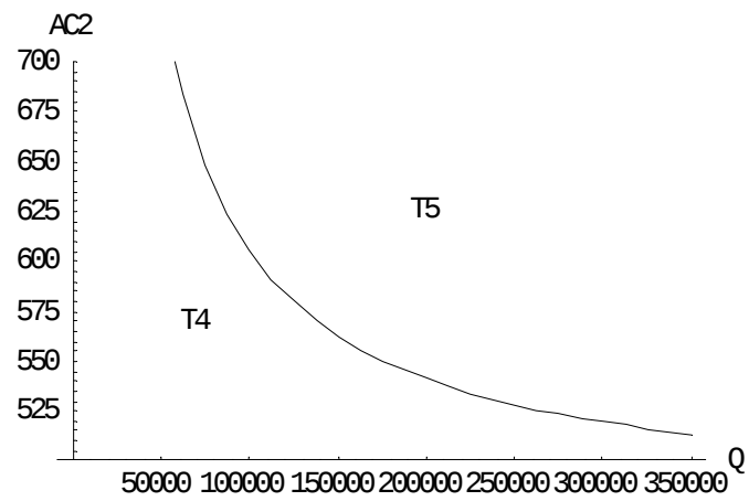
圖 6.6 貨物流量變動對船型決策之影響
