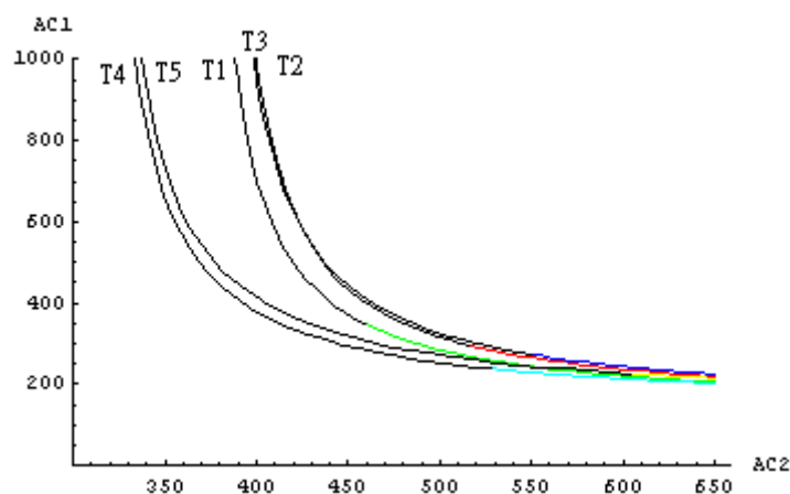
圖 6.4 各型船的可行解
