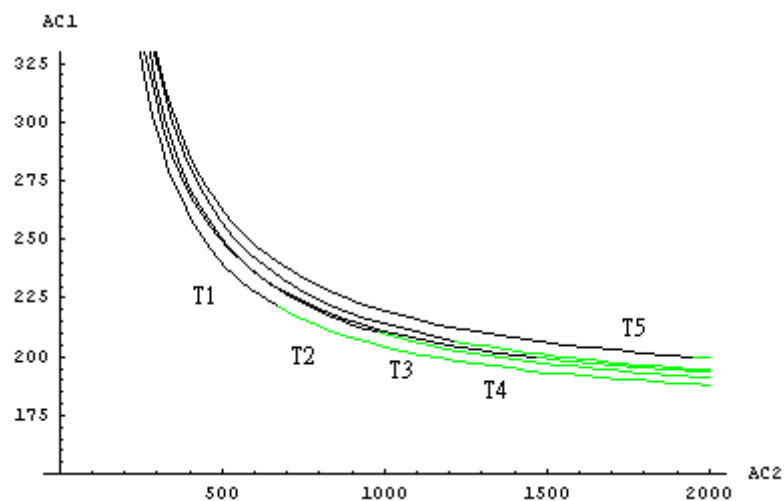
圖 8.5 胡志明港貨櫃經香港轉運之接駁航線的可行解
