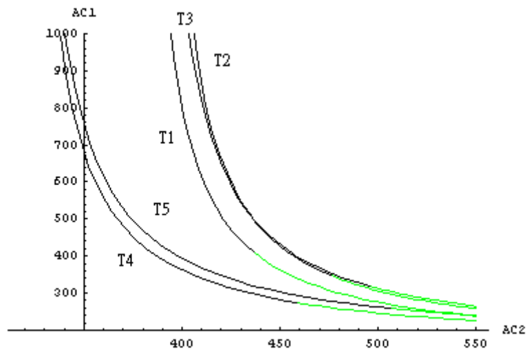
圖 7.2 馬尼拉港貨櫃經高雄港轉運之主航線的可行解
