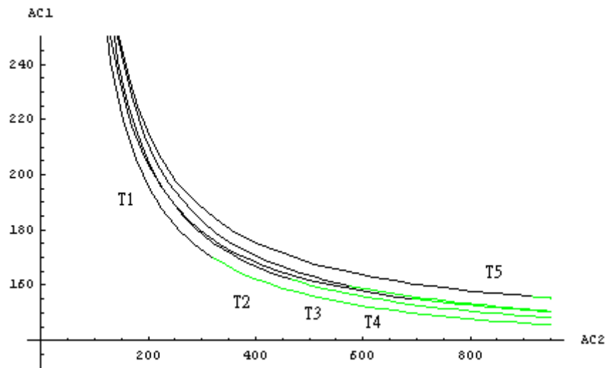
圖 7.3 馬尼拉港貨櫃經高雄港轉運之接駁航線的可行解
