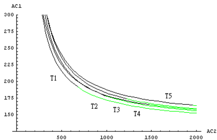
圖 8.3 胡志明港貨櫃經高雄港轉運之接駁航線的可行解
