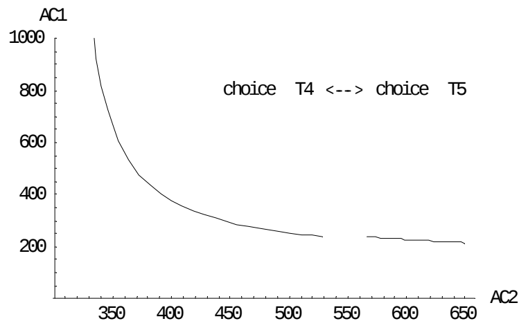
圖 6.5 TPN 航線之柏拉圖最佳解
