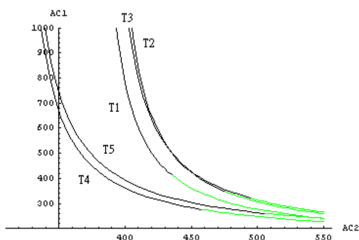
圖 7.4 馬尼拉港貨櫃經香港轉運之主航線的可行解
