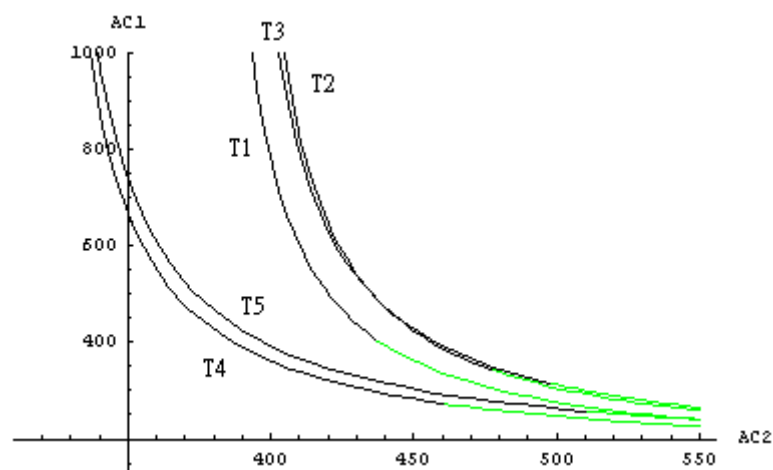
圖 8.2 胡志明港貨櫃經高雄港轉運之主航線的可行解
