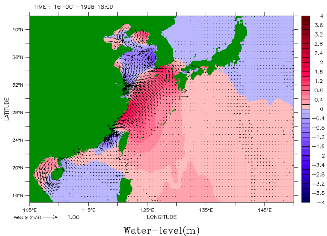
圖 4.2.1.2 瑞伯颱風期間平面流場截圖
