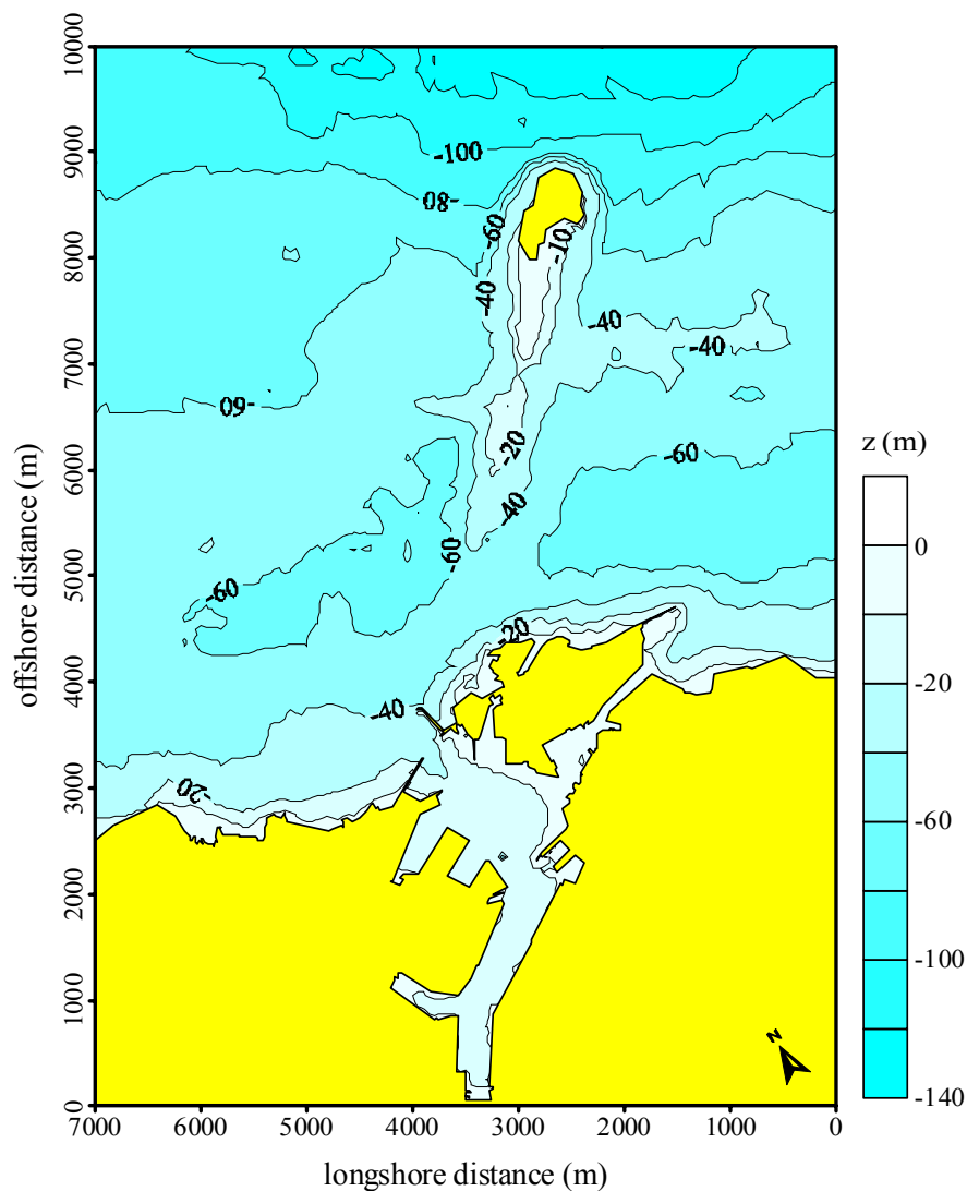
圖3.2.4 基隆港近岸區域波浪模式計算範圍及水深地形分佈圖
