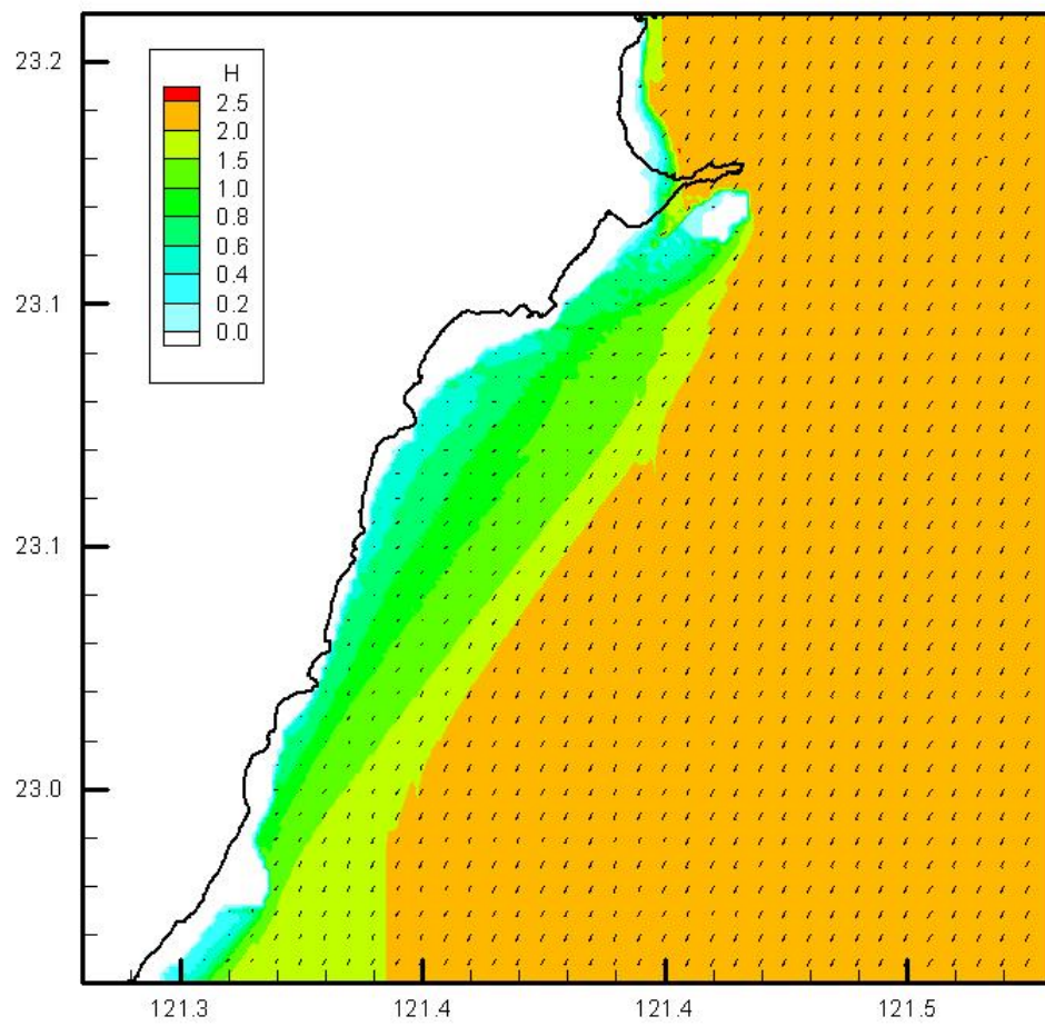
圖3.2.37 近岸區域波浪模式模擬區域K之波高及波向分佈
