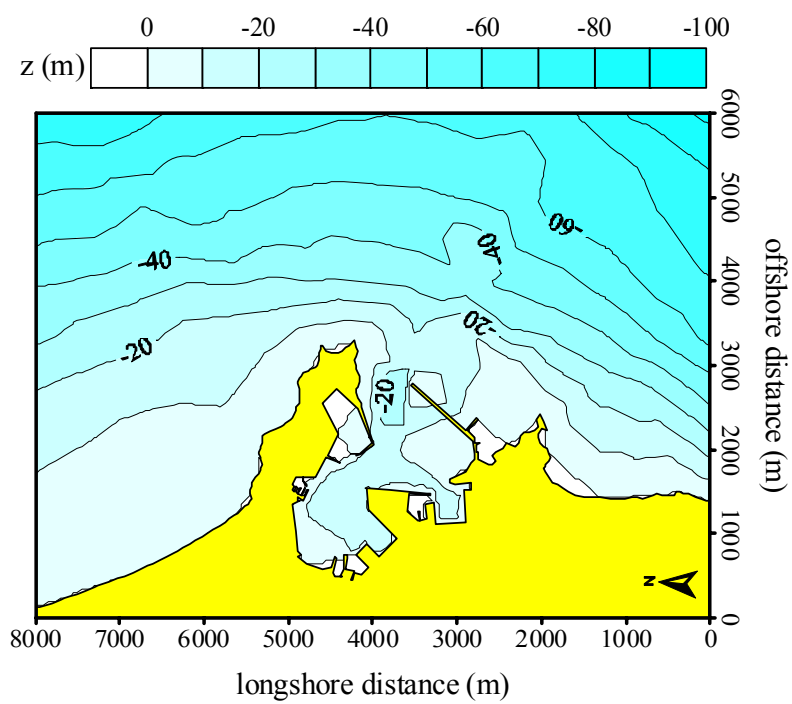
圖3.2.3 蘇澳港近岸區域波浪模式計算範圍及水深地形分佈圖
