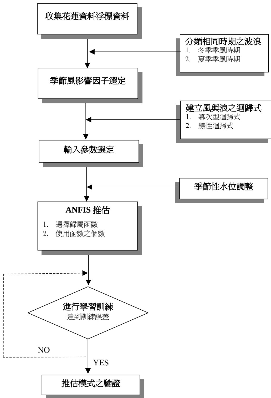
圖 3.3.25 模式建構流程圖
