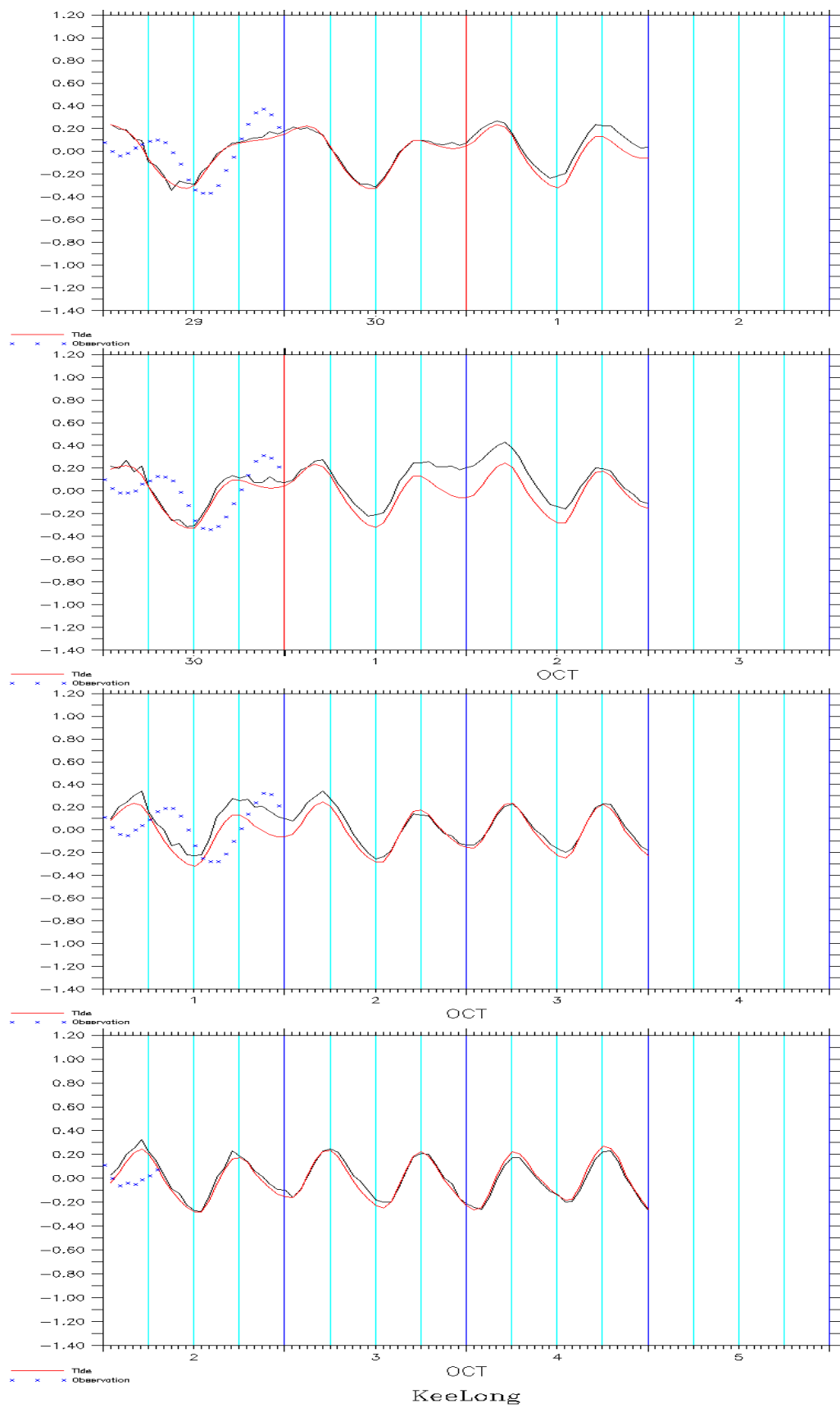
圖 6.2.21 龍王颱風期間基隆港水位預報圖（2005/09/30~10/03）
