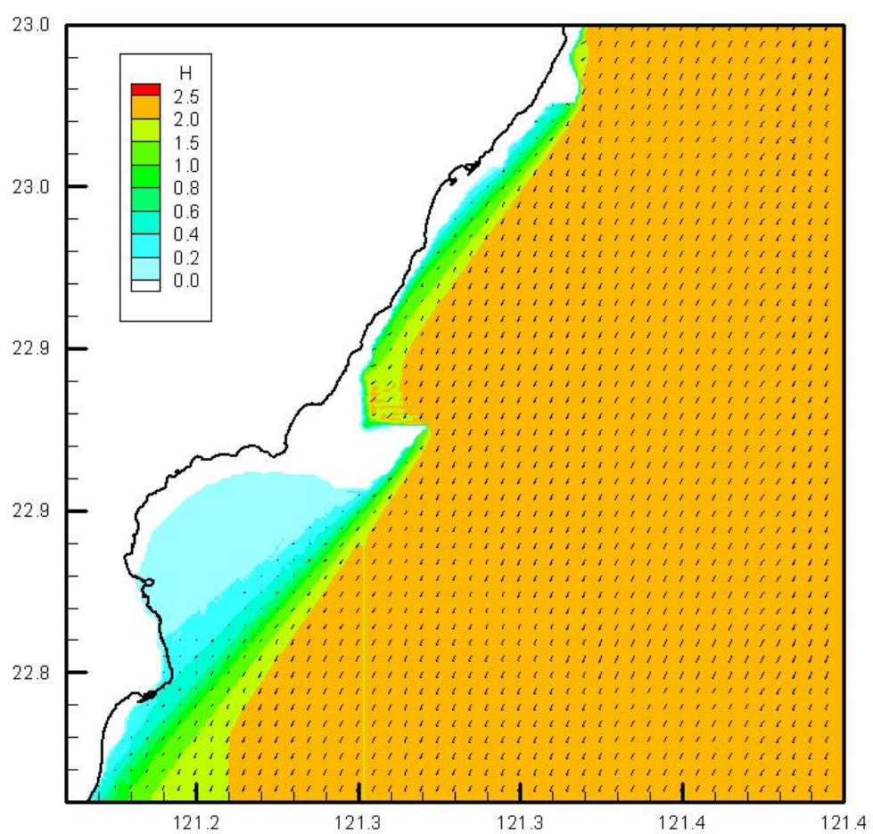
圖3.2.38 近岸區域波浪模式模擬區域L之波高及波向分佈
