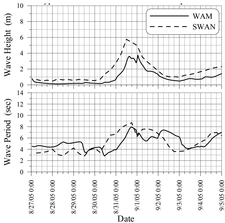
圖 3.1.18 泰利颱風侵襲時臺北港之推算波浪比較圖
