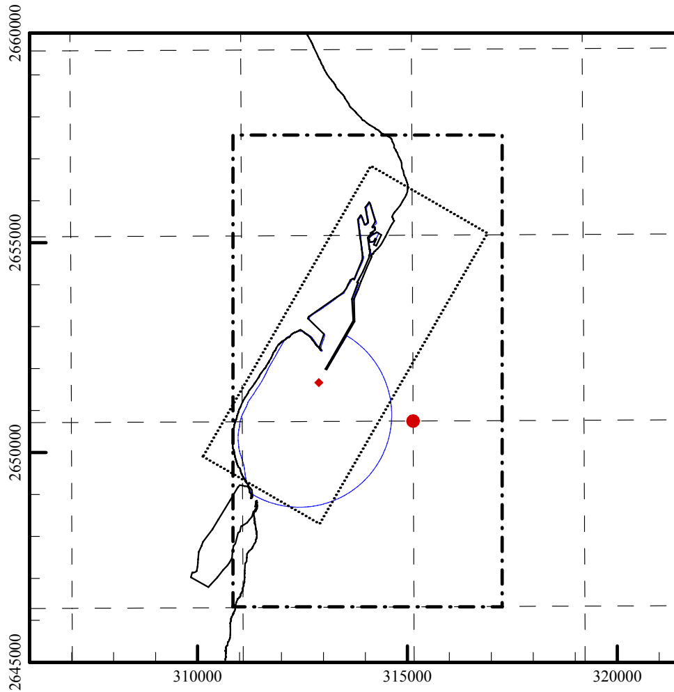
圖3.4.1 花蓮港波浪場相關數值模式模擬範圍示意圖(圖中虛線格網為全域SWAN模式計算網格，粗黑點虛線、點線及藍實線分別為區域模式、EEMSE模式及FEM EMS模式之計算範圍，圓形代表SWAN模式輸出點位，菱形代表波浪資料觀測位置)
