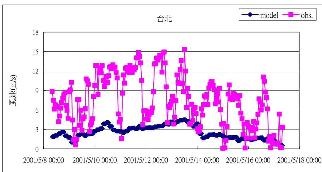
圖 2.1.14 西馬隆颱風期間模式風場與臺北實測資料比對圖
