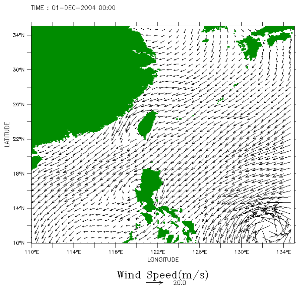
圖 2.2.3 中央氣象局 NFS 風場模式中國海域(15KM)風場向量圖
