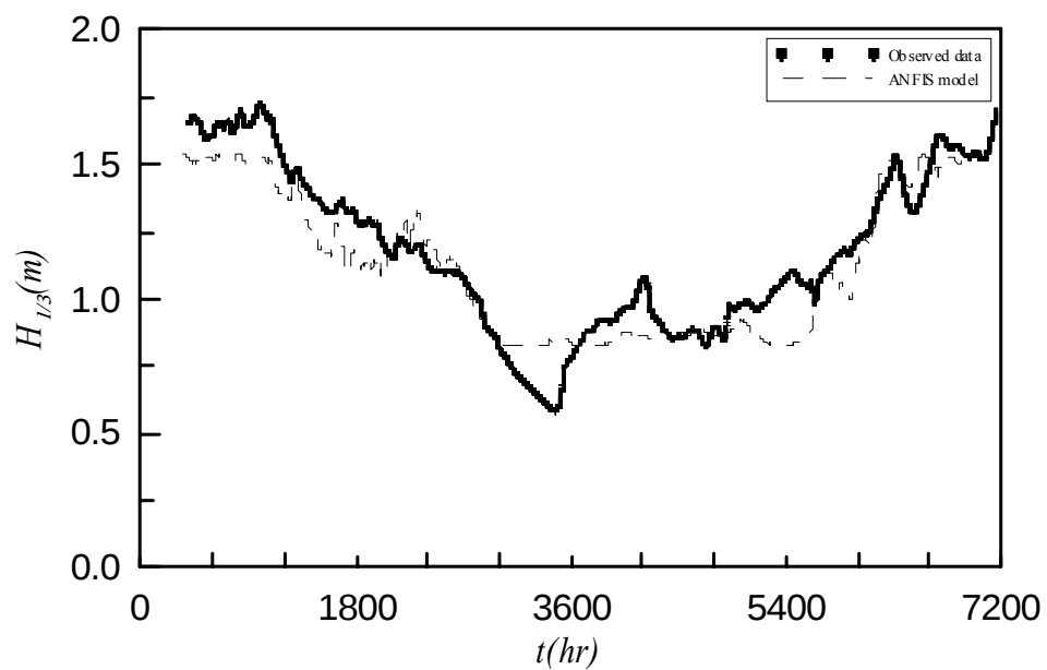
圖 3.3.31 以 2002 年之訓練輸出值與實際值的 720 小時之移動平均示性波高之比較圖
