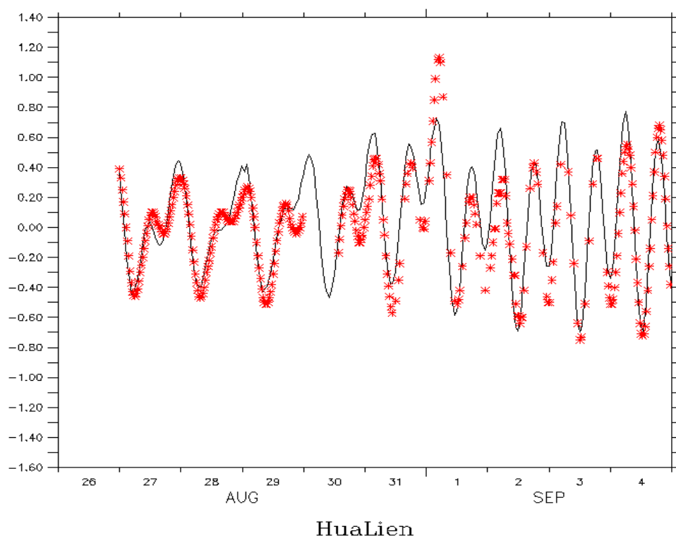
圖 4.1.1.9 泰利颱風期間花蓮測站水位比對圖
