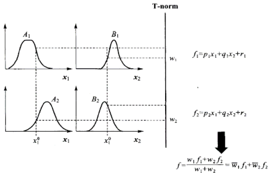
圖 3.3.22 Sugeno 模式示意圖
