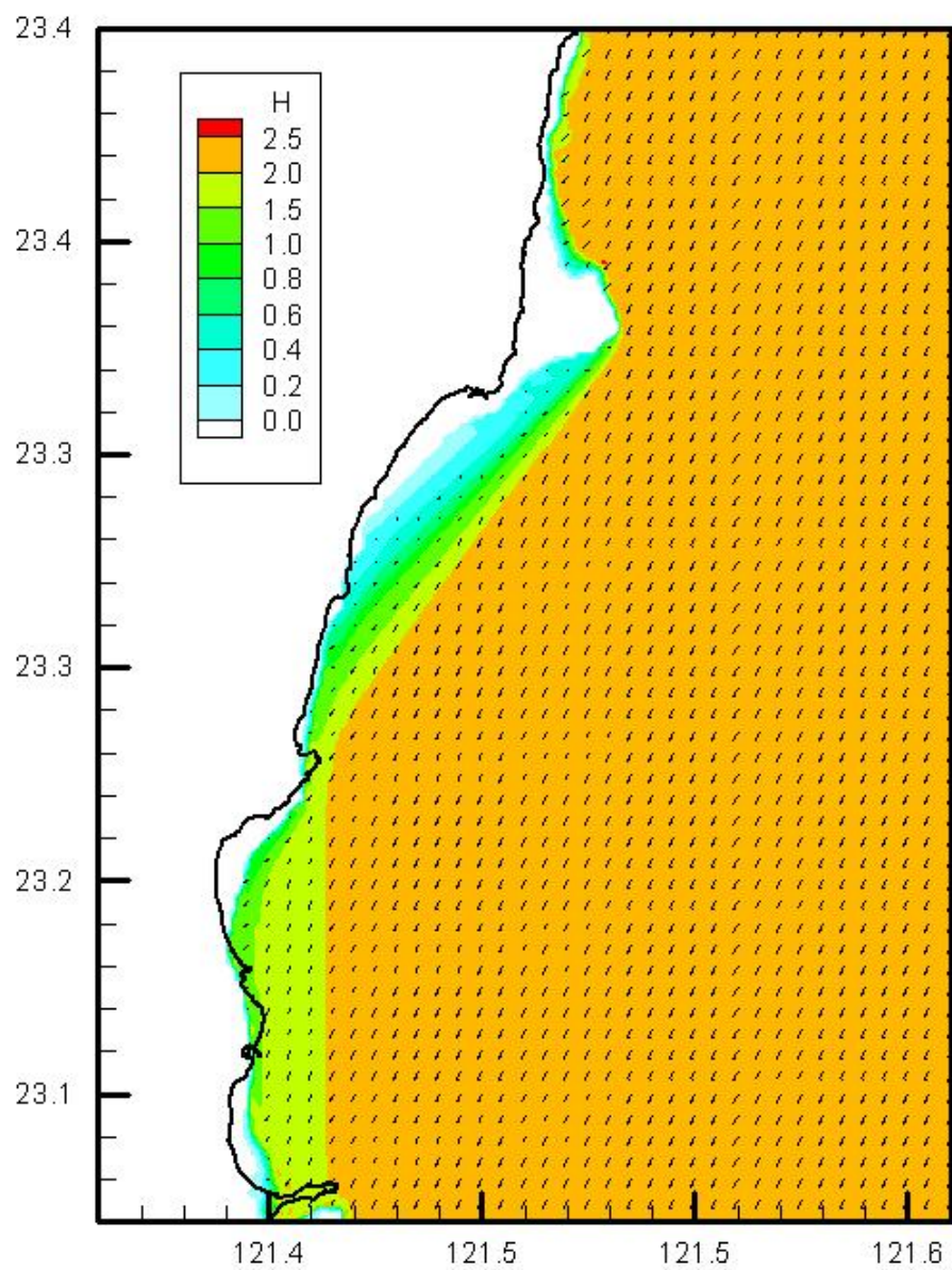
圖3.2.36 近岸區域波浪模式模擬區域J之波高及波向分佈
