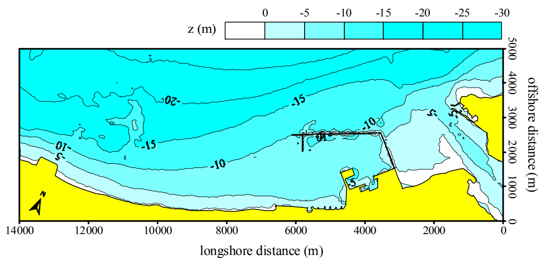
圖3.2.5 臺北港近岸區域波浪模式計算範圍及水深地形分佈圖
