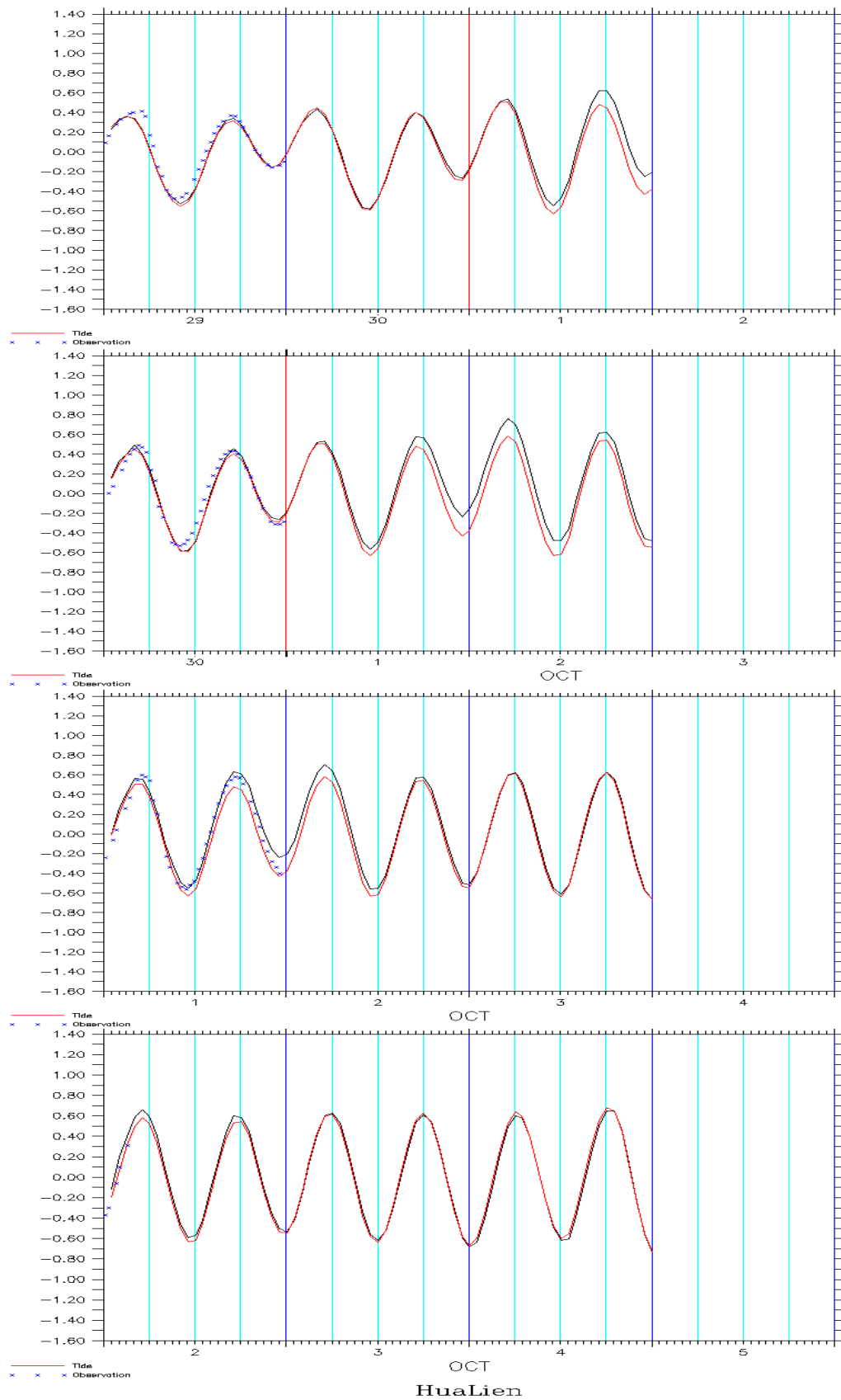
圖 6.2.20 龍王颱風期間花蓮港水位預報圖（2005/09/30~10/03）
