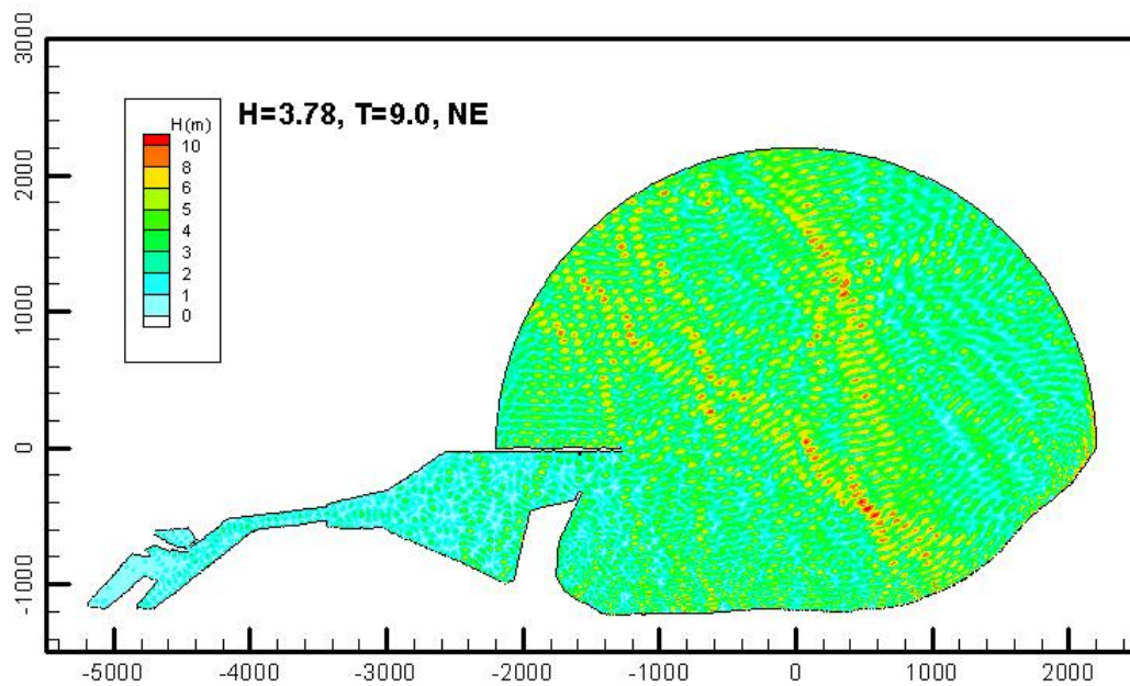
圖3.4.4 花蓮港近域波浪場之波高分布圖
