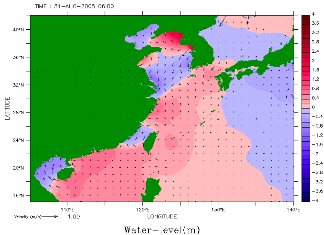
圖 4.2.2.3 泰利颱風期間底層流速分佈
