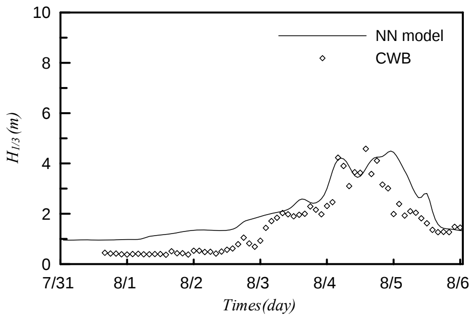
圖 3.3.7 蘇澳測站馬莎颱風神經網路模式推算與實測值比較
