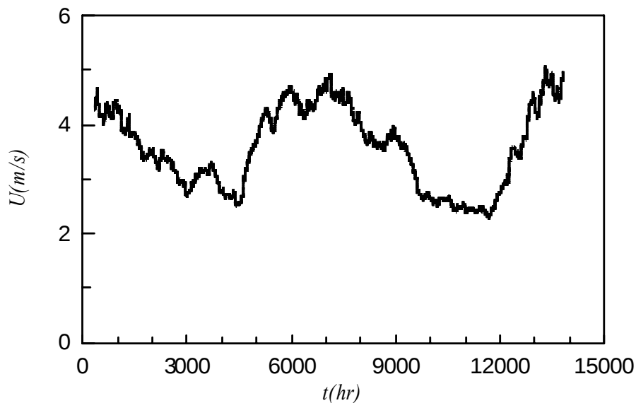
圖 3.3.26 2001-2002 花蓮站 720 小時之移動平均風速
