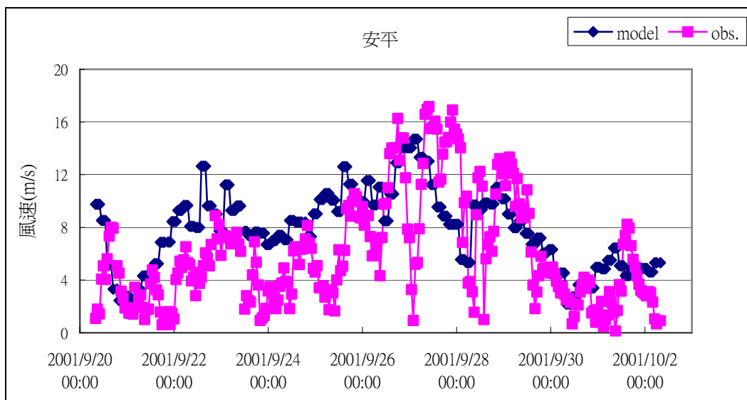
圖 2.1.7 利奇馬颱風期間模式風場與安平實測資料比對圖
