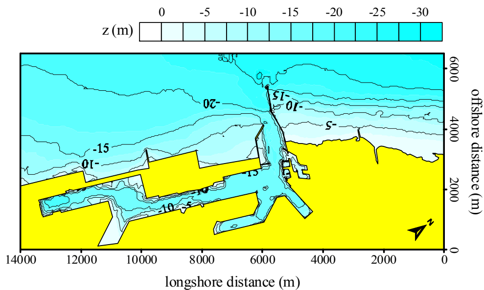
圖3.2.6 臺中港近岸區域波浪模式計算範圍及水深地形分佈圖
