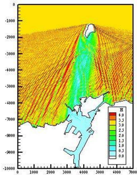
圖3.2.13 基隆港近岸波浪場模擬結果(a)EEMSE近域模式(b) REF/DIF 區域模式(艾莉颱風， H=3.40\text{m} ， T=8.61\text{sec} ， E20.9^\circ\text{N} )
