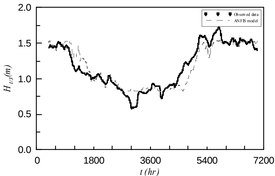
圖 3.3.29 以 2001 年之訓練輸出值與實際值的 720 小時之移動平均示性波高之比較圖
