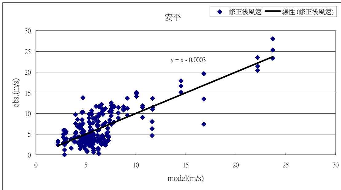
圖 2.1.16 桃芝颱風期間修正後之模式風場與安平實測資料趨勢圖
