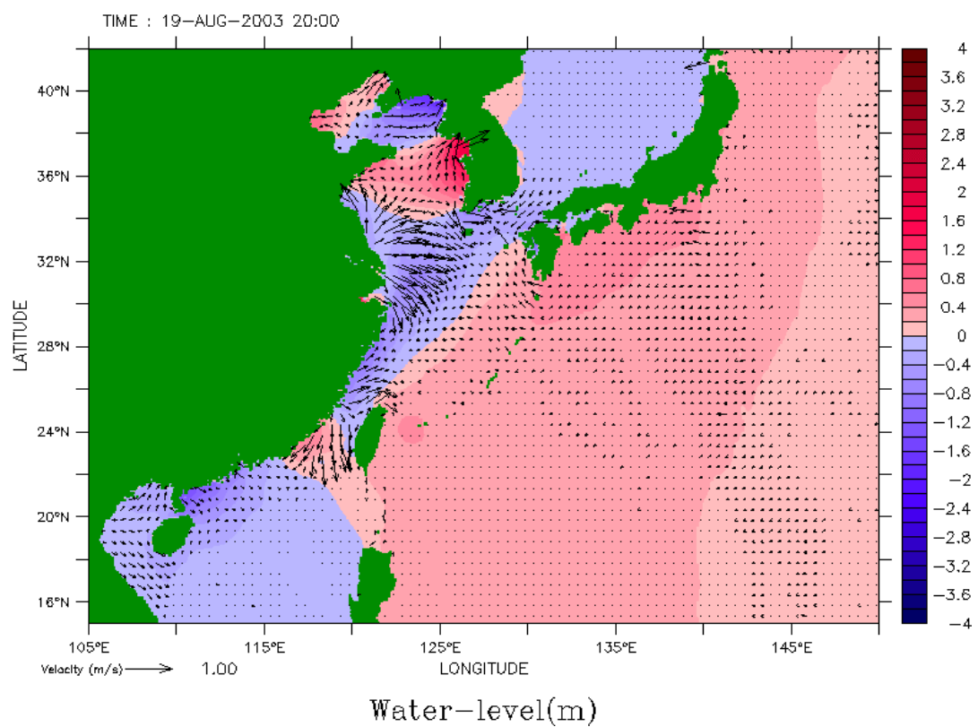
圖 4.2.1.7 梵高颱風期間平面流場截圖
