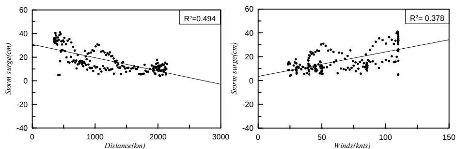
圖4.1.2.9 雷馬遜颱風暴潮偏差與測站距離及中心風速相關性分析
