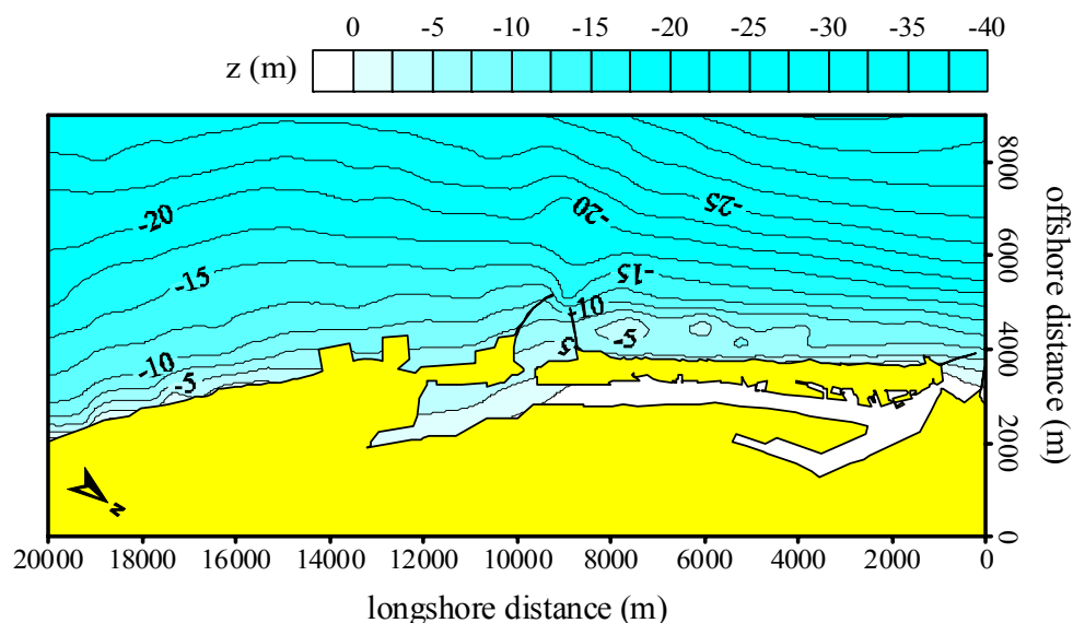
圖3.2.8 高雄港近岸區域波浪模式計算範圍及水深地形分佈圖
