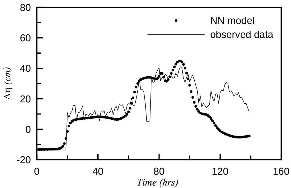
圖 4.1.2.18 蘭寧颱風暴潮偏差與觀測值比較
