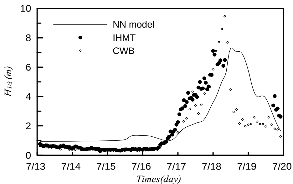
圖 3.3.4 花蓮測站海棠颱風神經網路模式推算與實測值比較
