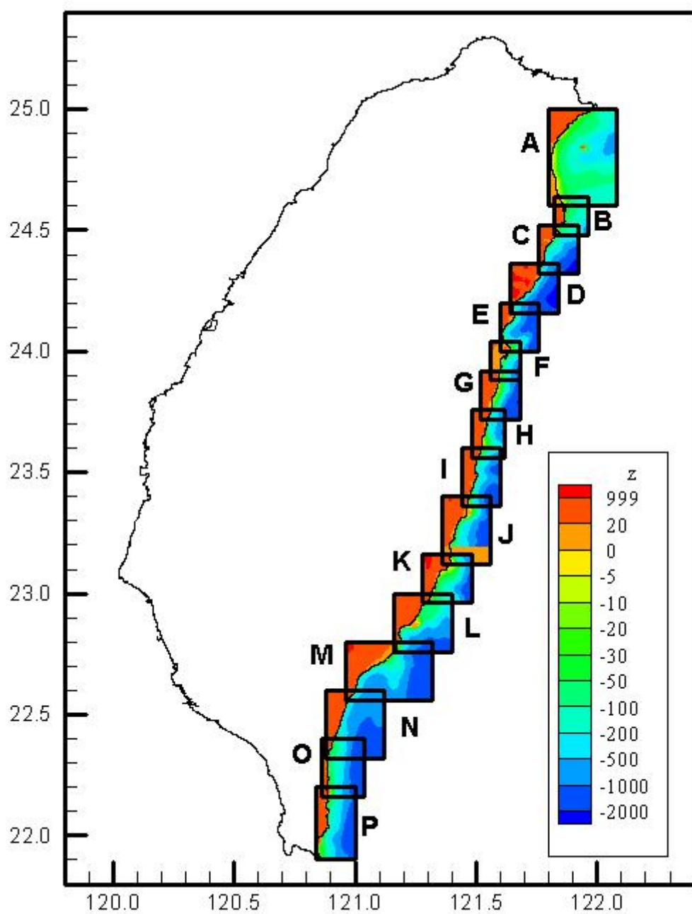
圖3.2.24 臺灣東部海岸近岸區域波浪模式模擬範圍示意圖
