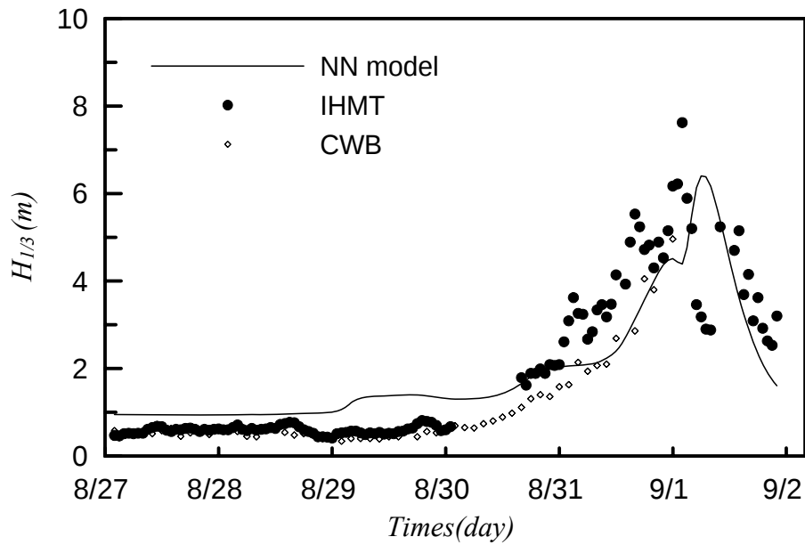
圖 3.3.10 花蓮測站泰利颱風神經網路模式推算與實測值比較
