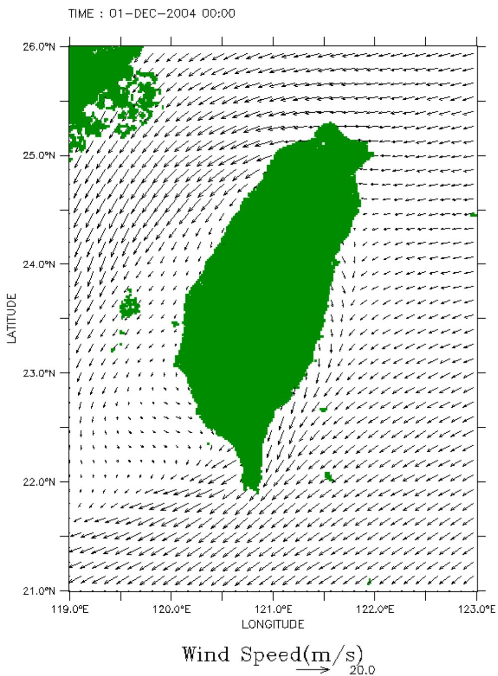
圖 2.2.4 中央氣象局 NFS 風場模式臺灣海域(5KM)風場向量圖
