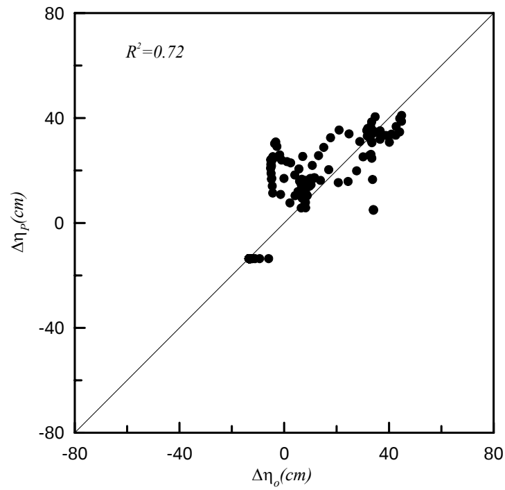
圖 4.1.2.17 蘭寧颱風類神經網路模式測試結果關係圖
