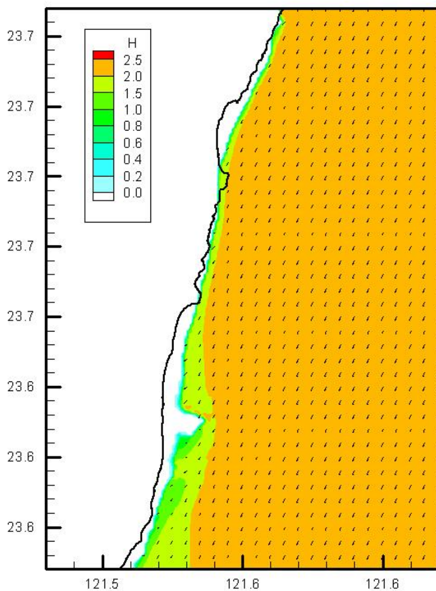
圖3.2.34 近岸區域波浪模式模擬區域H之波高及波向分佈
