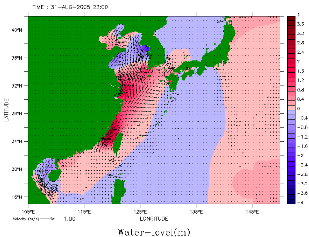
圖 4.2.1.12 泰利颱風期間平面流場截圖
