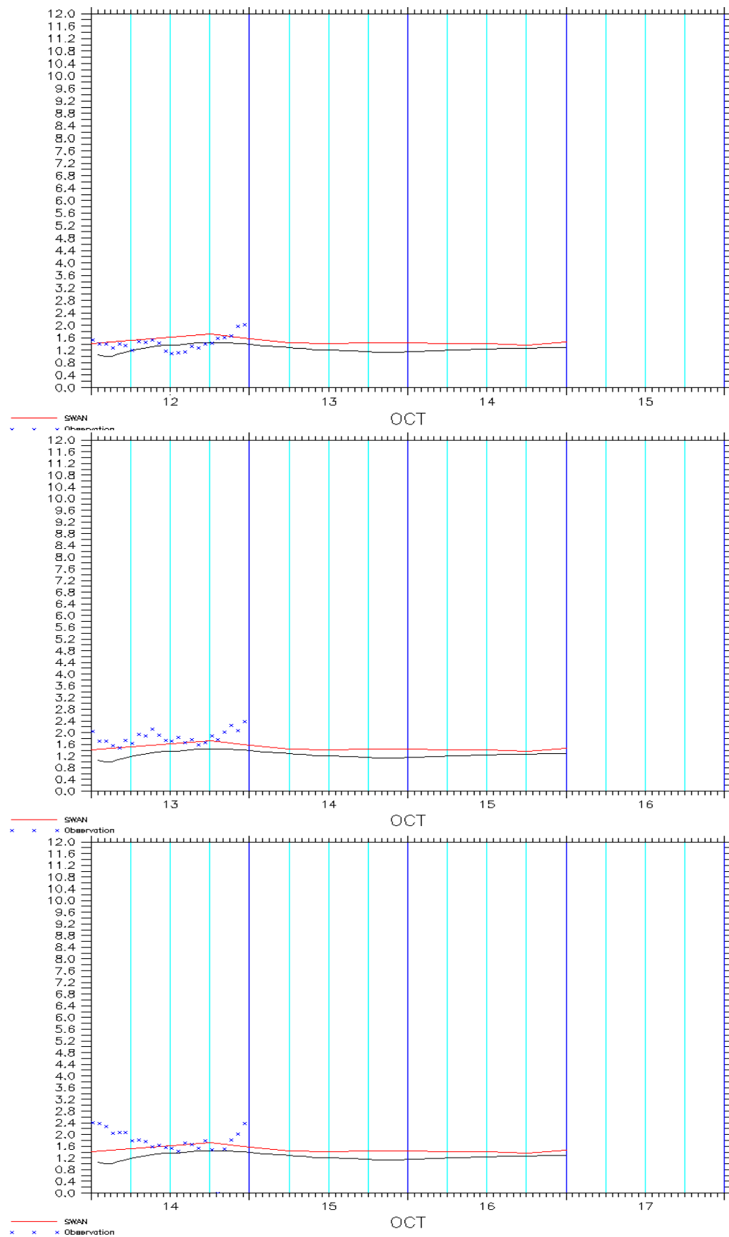
圖 6.2.34 非颱風期間蘇澳港波高預報圖 (2005/10/13~15)
