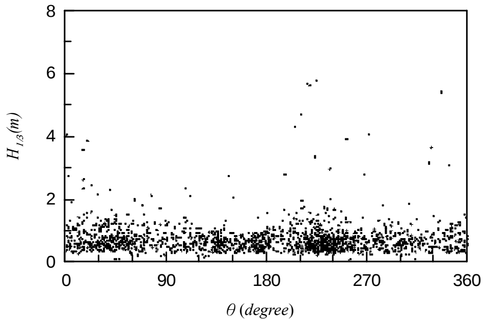
圖 3.3.21 2002 年夏季季風時期風向與示性波高關係
