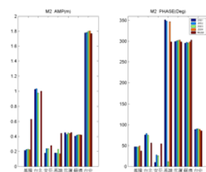
圖4.1b 各港口M2調和常數比較 (實測與天文潮模式)
