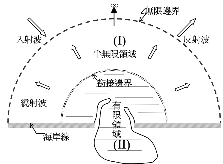
圖3.4.2 任意水深港域波浪場示意圖
