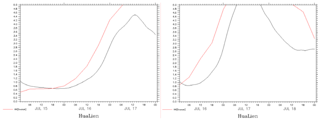
圖 6.2.11 海棠颱風期間花蓮波浪預報圖（2005/07/16~07/17）
