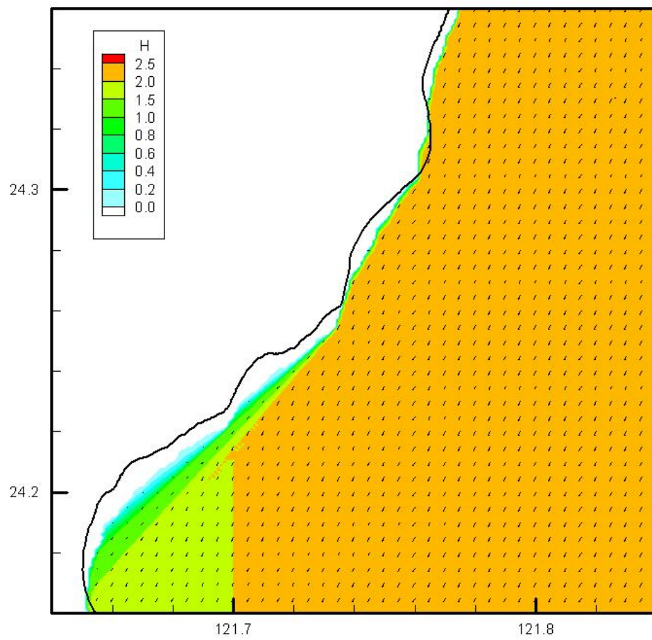
圖3.2.30 近岸區域波浪模式模擬區域D之波高及波向分佈
