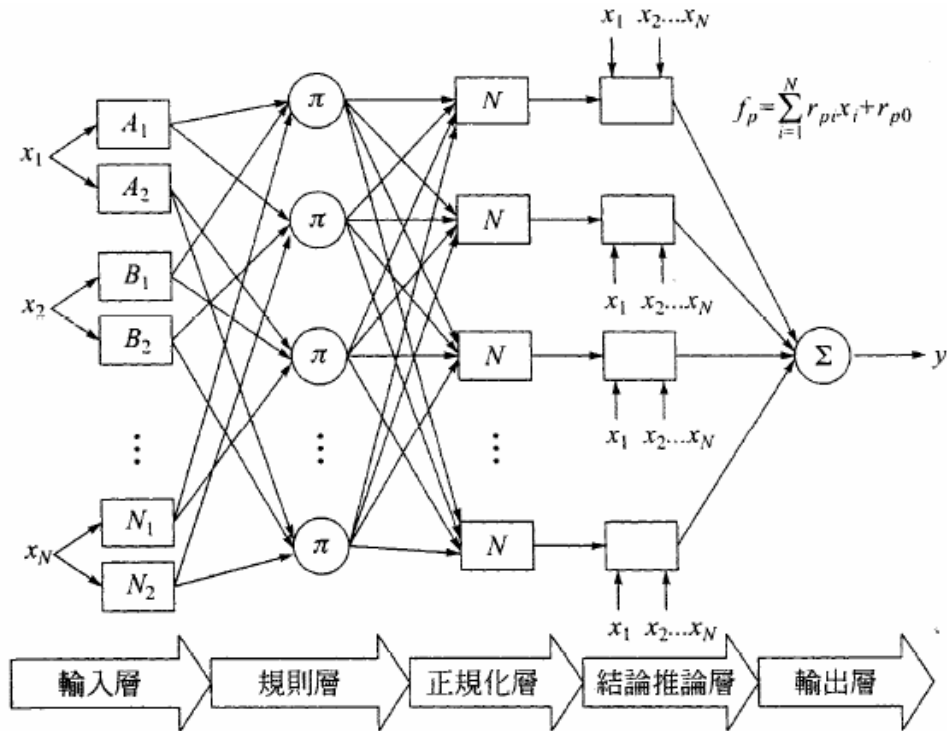
圖 3.3.24 適應性網路架構模糊推論系統架構示意圖
