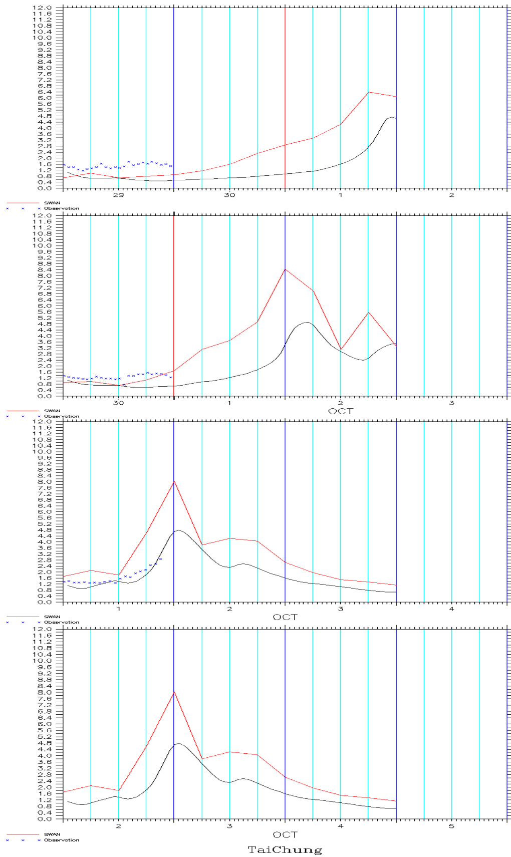
圖 6.2.27 龍王颱風期間臺中港波高預報圖（2005/09/30~10/03）
