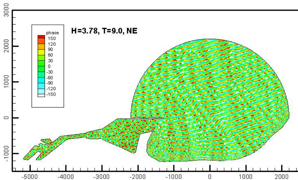
圖3.4.5 花蓮港近域波浪場之相位分布圖
