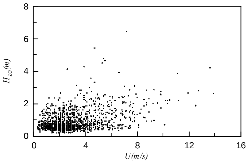
圖 3.3.16 2001 年夏季季風時期風速與示性波高關係
