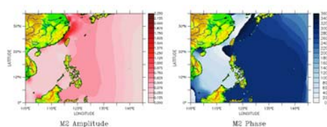
圖4.1a M2分潮振幅與遲角(大尺度) (天文潮模式)
