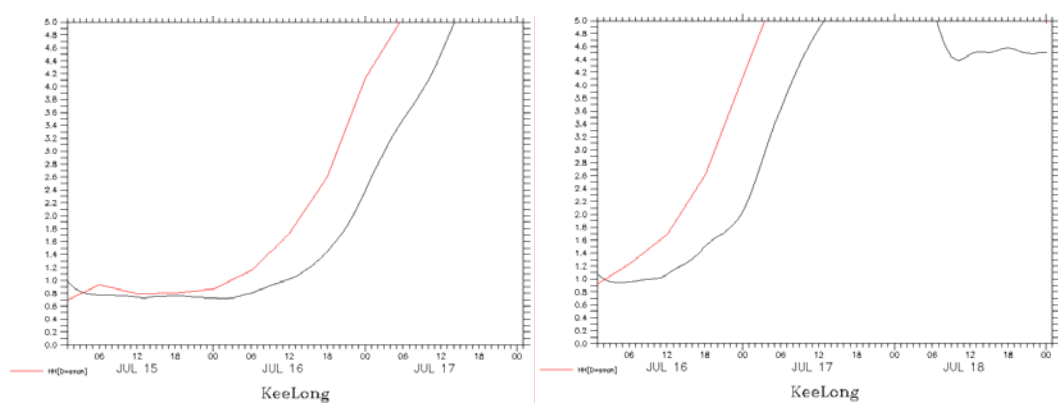
圖 6.2.12 海棠颱風期間基隆波浪預報圖（2005/07/16~07/17）
