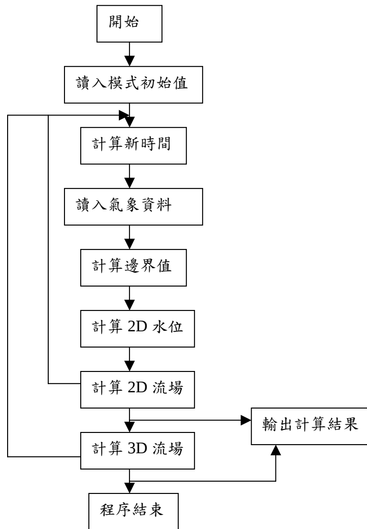
圖 4.1.1.4 COHERENS 計算流程
