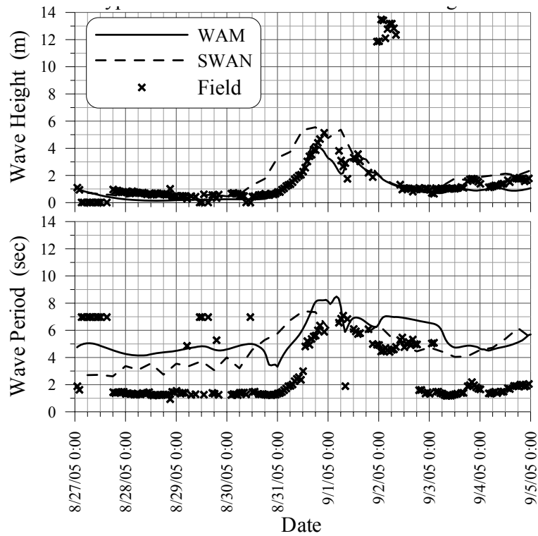
圖 3.1.15 泰利颱風侵襲時臺中港之推算波浪與觀測波浪比較圖
