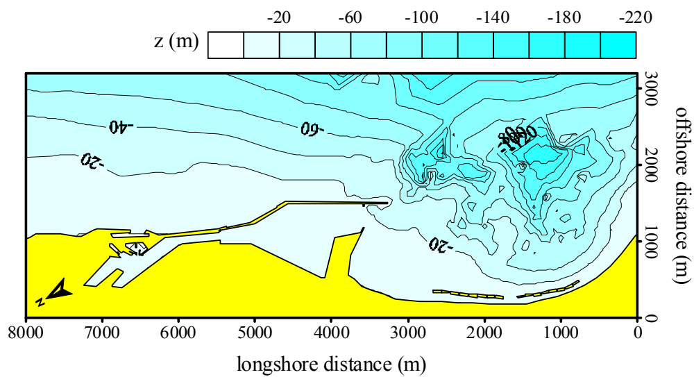
圖3.2.2 花蓮港近岸區域波浪模式計算範圍及水深地形分佈圖
