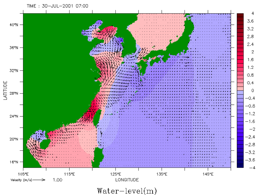
圖 4.2.1.5 桃芝颱風期間平面流場截圖
