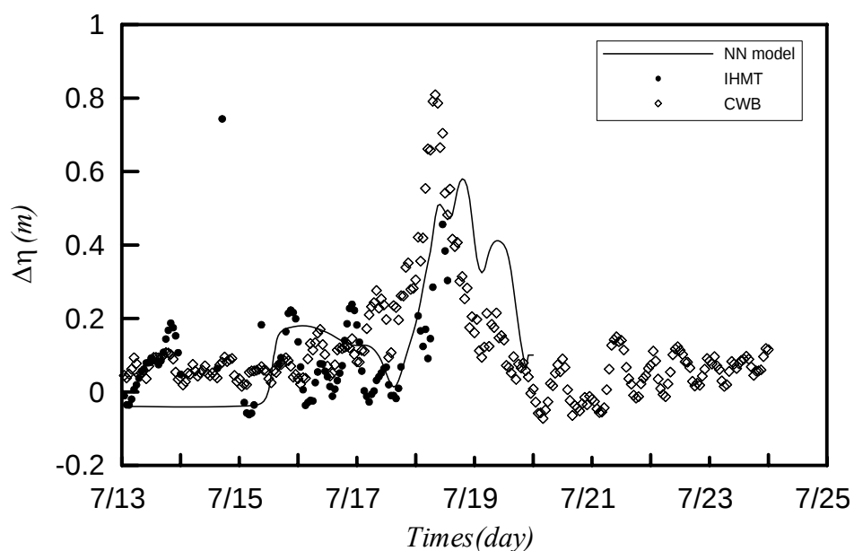
圖 4.1.2.21 海棠颱風暴潮偏差與蘇澳港觀測值之比較
