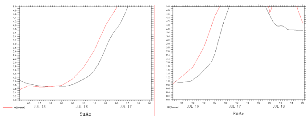
圖 6.2.13 海棠颱風期間蘇澳波浪預報圖（2005/07/16~07/17）
