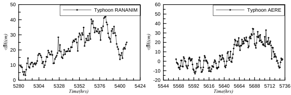
圖4.1.2.3 蘭寧（RANANIM）與艾利（AERE）之暴潮偏差
