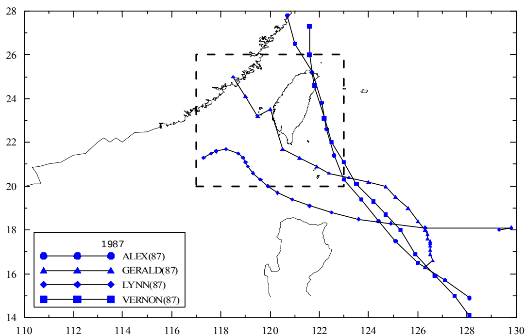
圖 3.5.2 (續 9)歷年侵臺颱風路徑圖 (1987 年)
