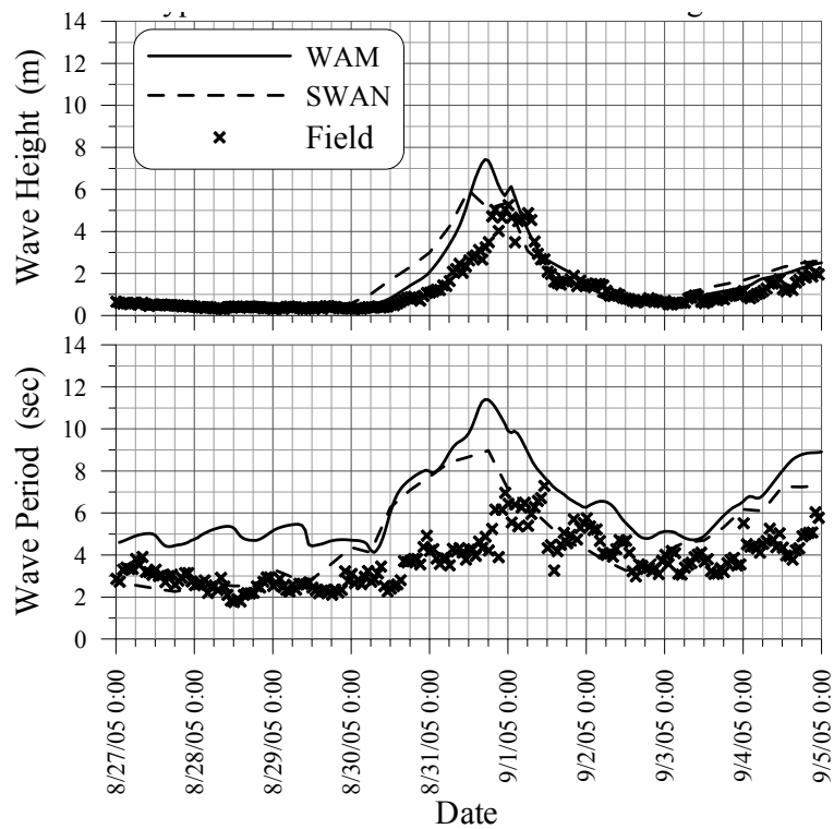
圖 3.1.14 泰利颱風侵襲時基隆港之推算波浪與觀測波浪比較圖
