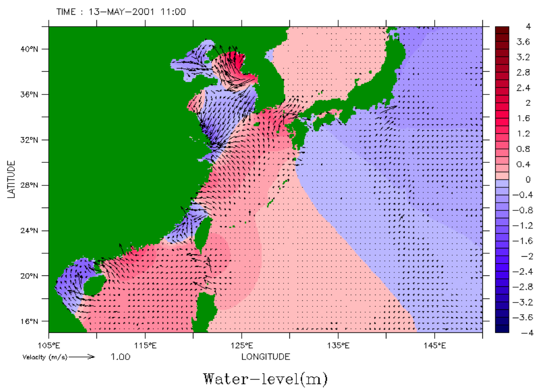
圖 4.2.1.3 西馬隆颱風期間平面流場截圖
