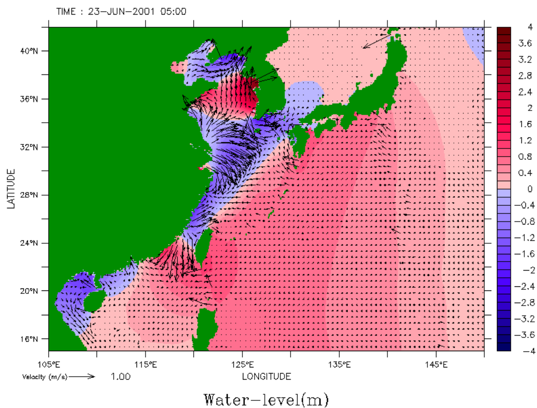
圖 4.2.1.4 奇比颱風期間平面流場截圖
