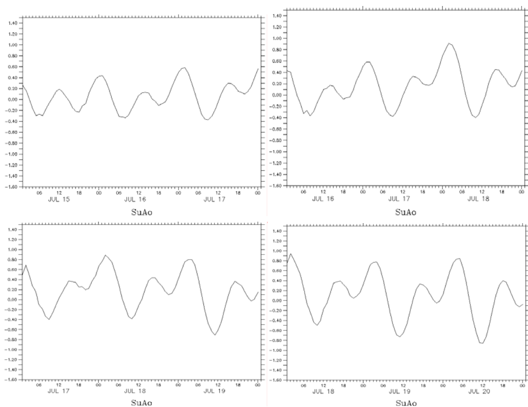
圖 6.2.9 海棠颱風期間蘇澳港水位預報圖（2005/07/16~07/19）
