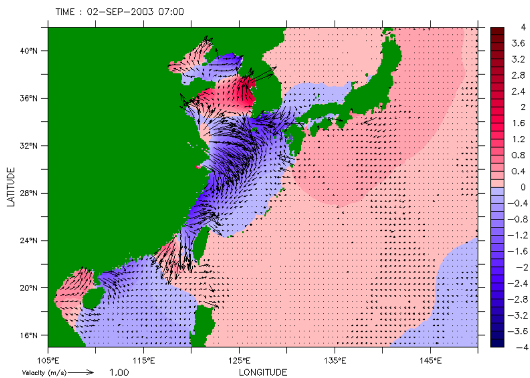
圖 4.2.1.8 杜鵑颱風期間平面流場截圖
