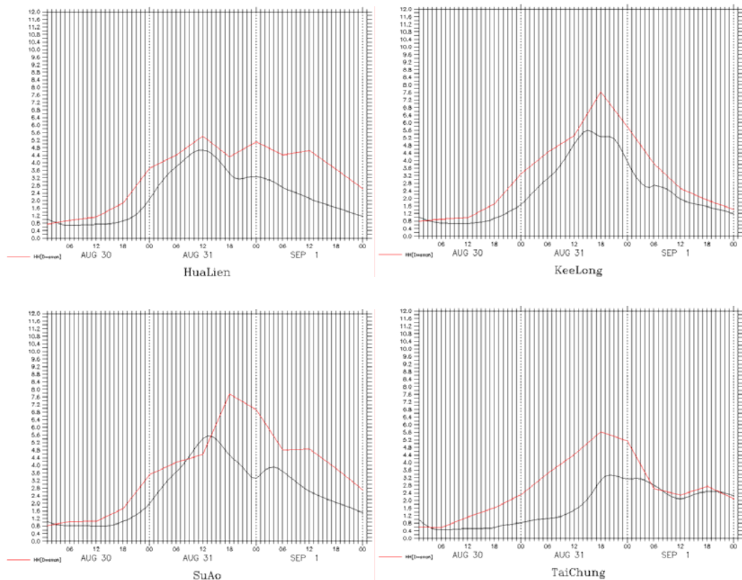
圖 6.2.19 泰利颱風期間波浪預報圖（2005/08/31）
