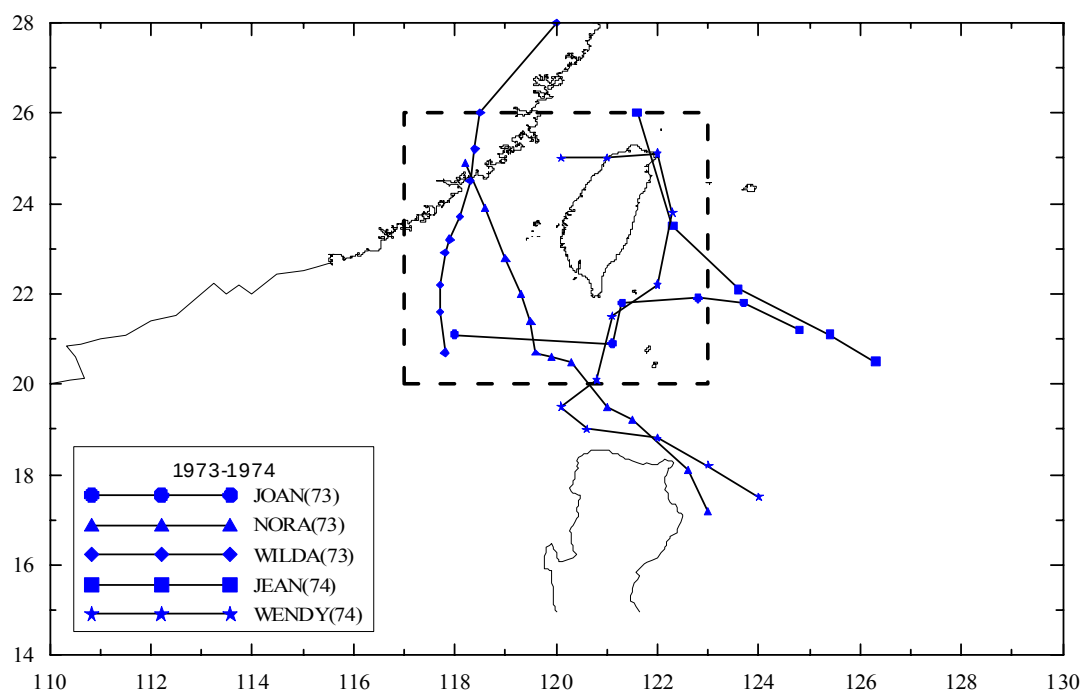
圖 3.5.2 (續 1) 歷年侵臺颱風路徑圖 (1973-1974 年)
