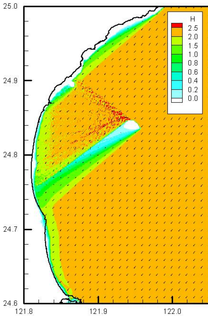
圖3.2.27 近岸區域波浪模式模擬區域A之波高及波向
