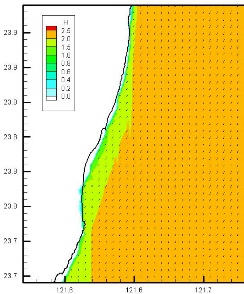
圖3.2.33 近岸區域波浪模式模擬區域G之波高及波向分佈
