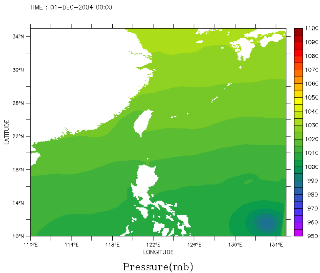
圖 2.3.2 中央氣象局 NFS 風壓模式中國海域(15KM)等氣壓圖
