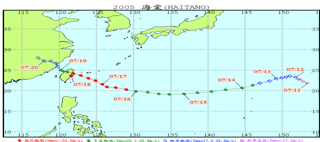
圖 3.1.5 2005 年 7 月海棠(Haitang)颱風記錄與路徑圖
