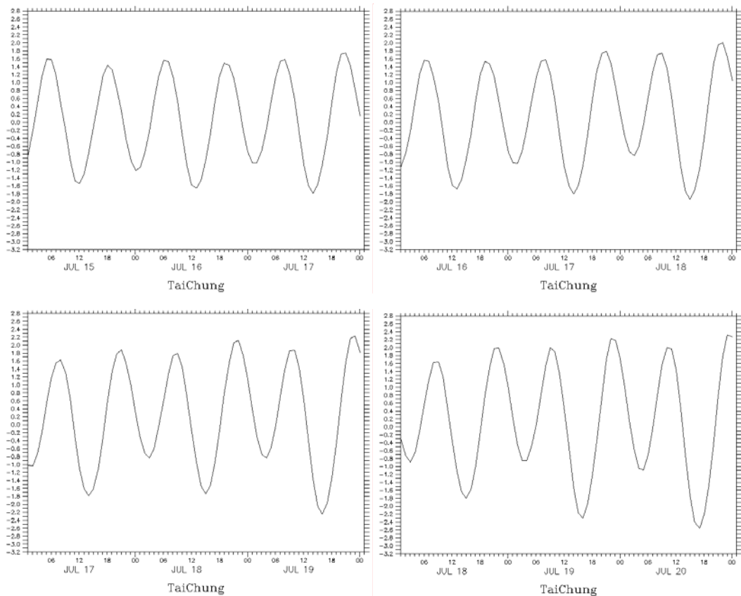
圖 6.2.10 海棠颱風期間臺中港水位預報圖（2005/07/16~07/19）
