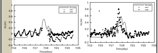
海棠颱風花蓮測站暴潮預測值
