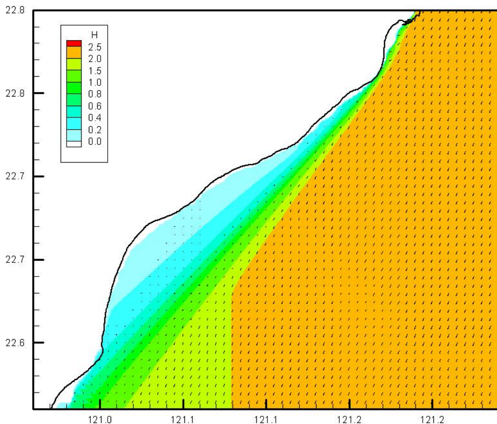
圖 3.2.39 近岸區域波浪模式模擬區域 M 之波高及波向分佈
