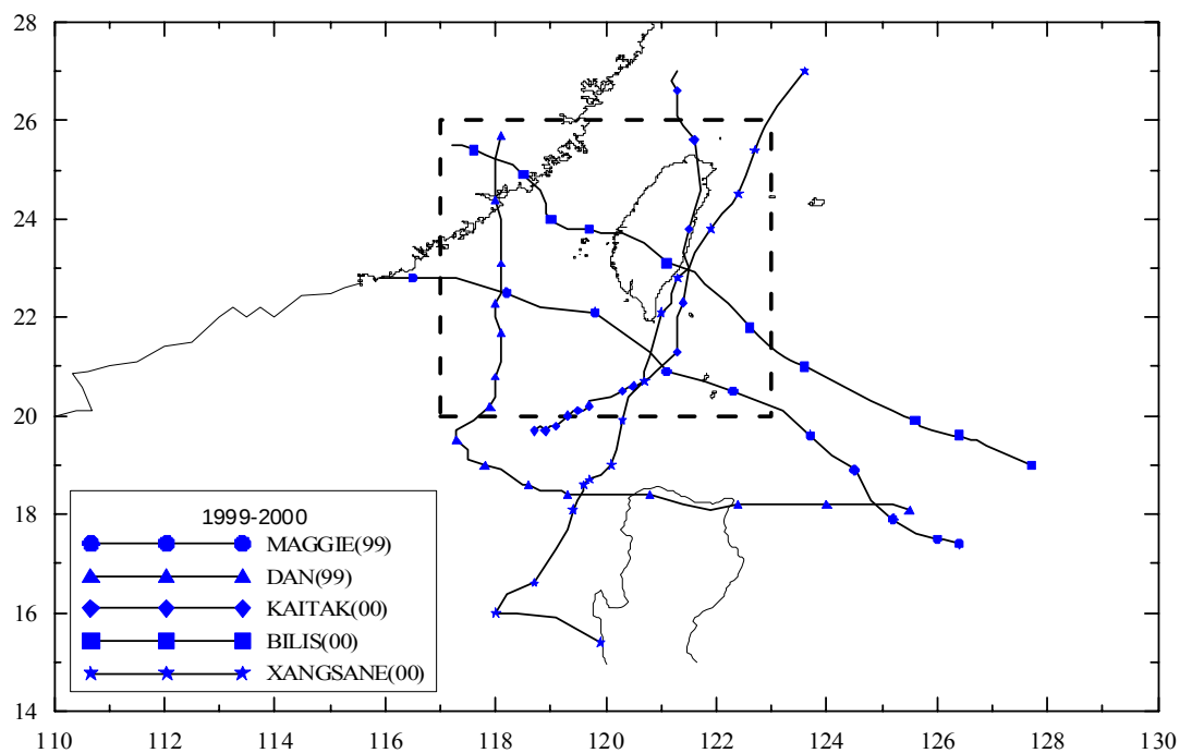
圖 3.5.2 (續 16)歷年侵臺颱風路徑圖 (1999-2000 年)
