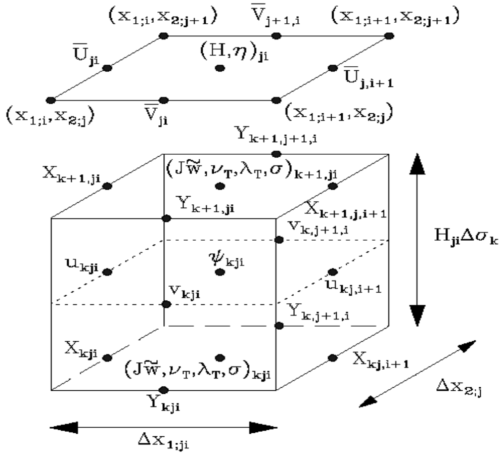
圖 4.1.1.1 二維及三維的格點分佈
