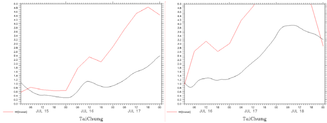
圖 6.2.14 海棠颱風期間臺中波浪預報圖（2005/07/16~07/17）
