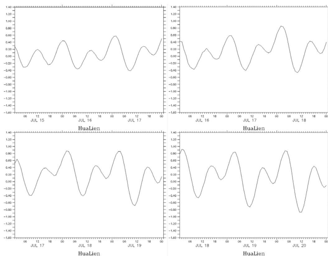
圖 6.2.7 海棠颱風期間花蓮港水位預報圖（2005/07/16~07/19）
