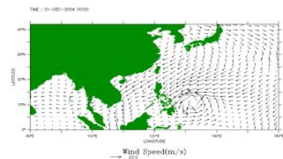
圖2.2a 中央氣象局NFS風場模式西太平洋(45KM)風場向量圖
