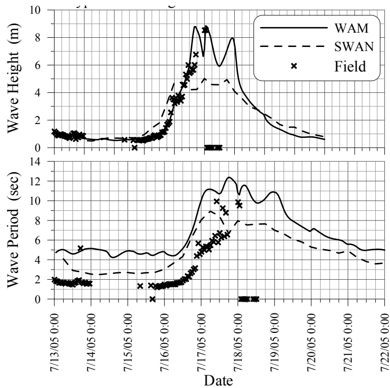
圖 3.1.8 海棠颱風侵襲時蘇澳港之推算波浪與觀測波浪比較圖
