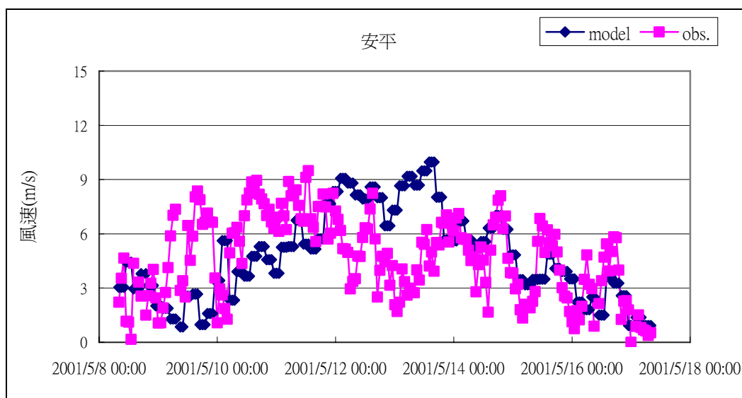
圖 2.1.13 西馬隆颱風期間模式風場與安平實測資料比對圖
