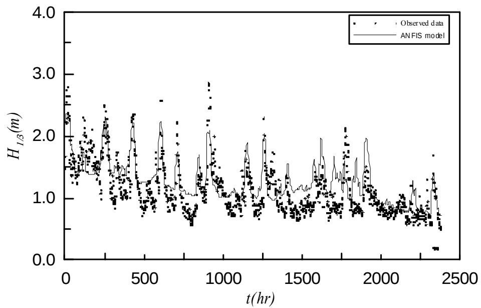
圖 3.3.39 2002 年 1-4 月實測與推算波高時序圖
