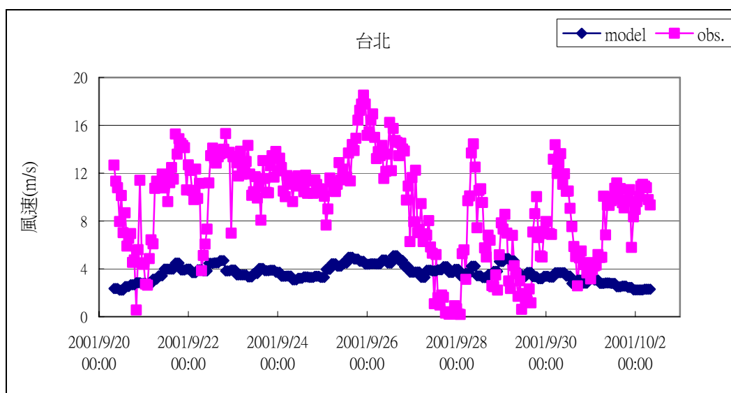
圖 2.1.8 利奇馬颱風期間模式風場與臺北實測資料比對圖
