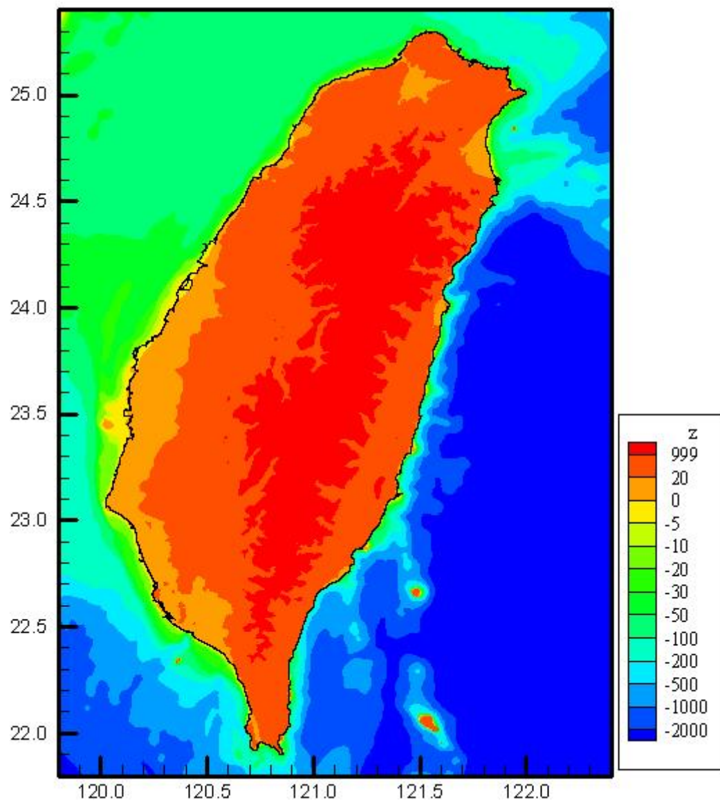
圖3.2.23 臺灣環島海域地形水深圖
