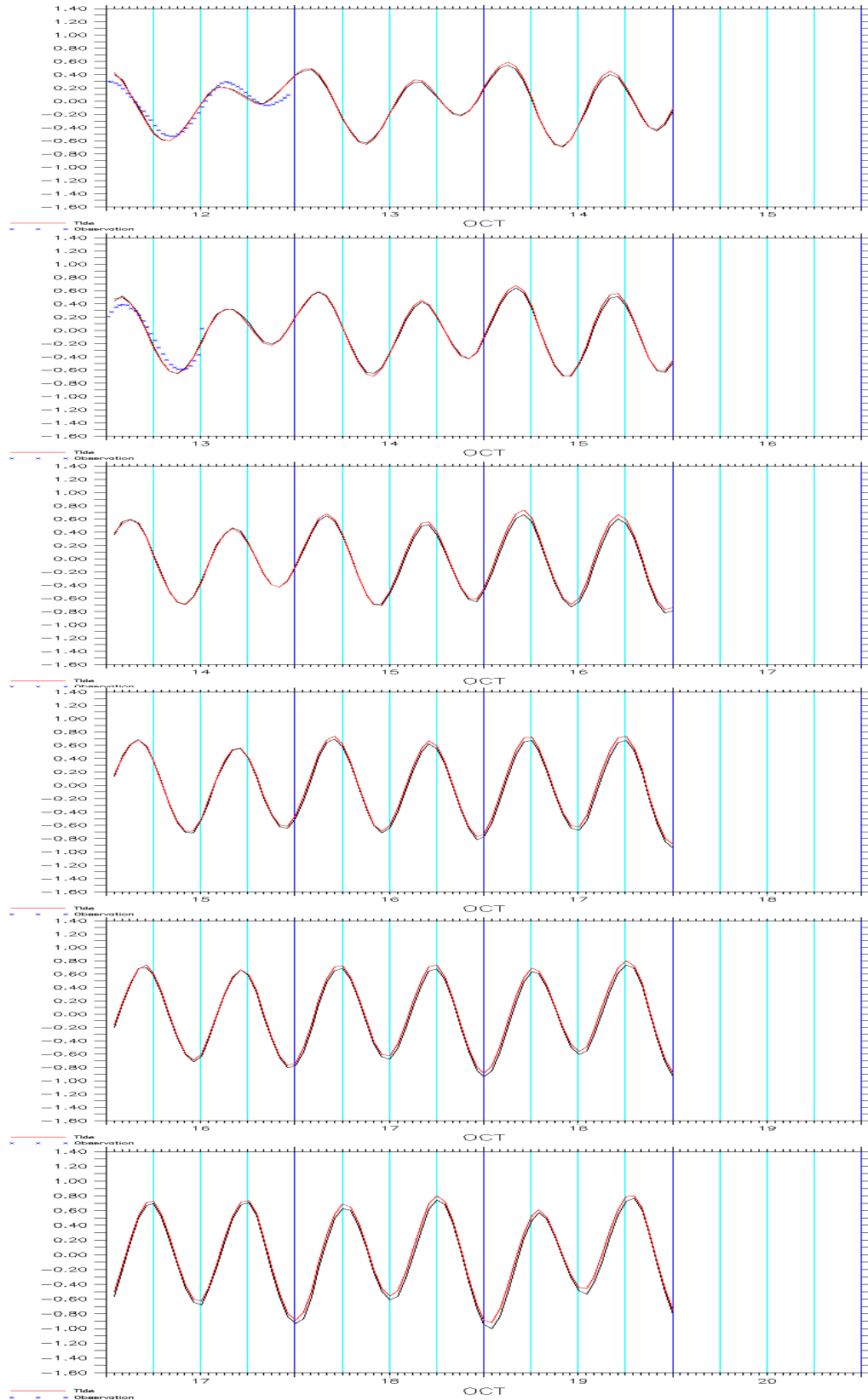
圖 6.2.28 非颱風期間花蓮港水位預報圖（2005/10/13~18）
