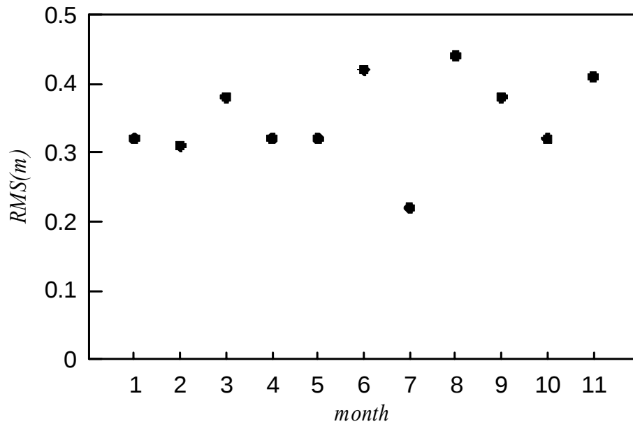
圖 3.3.45 2002 年各月份之推估波高 RMS 值
