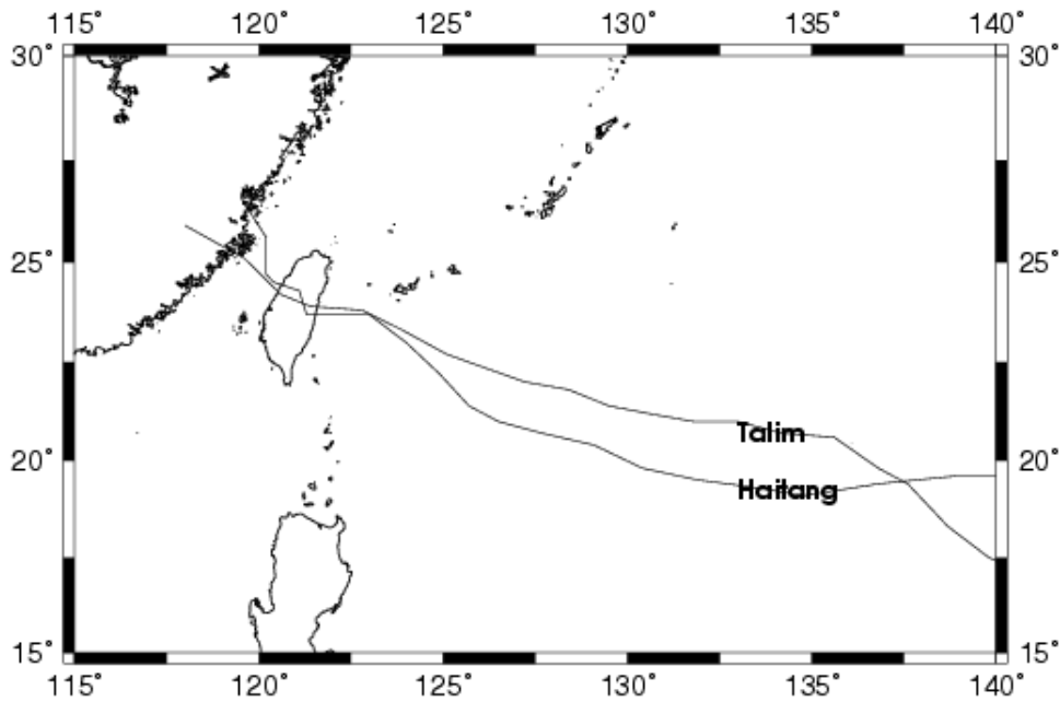
圖 4.1.2.19 海棠及泰利颱風行進路徑圖
