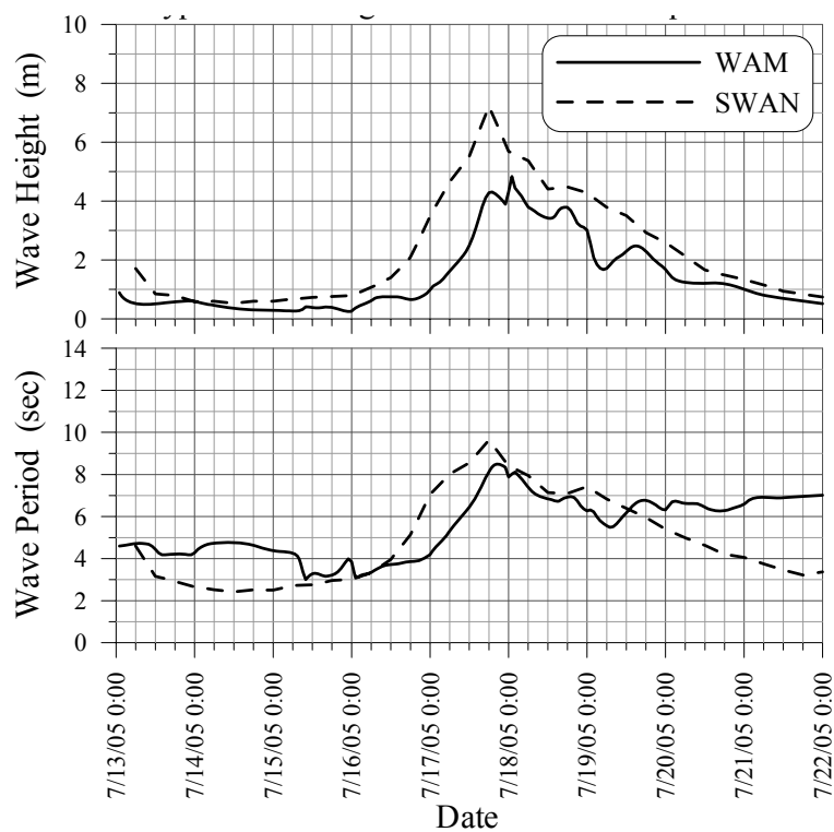
圖 3.1.10 海棠颱風侵襲時臺北港之推算波浪比較圖
