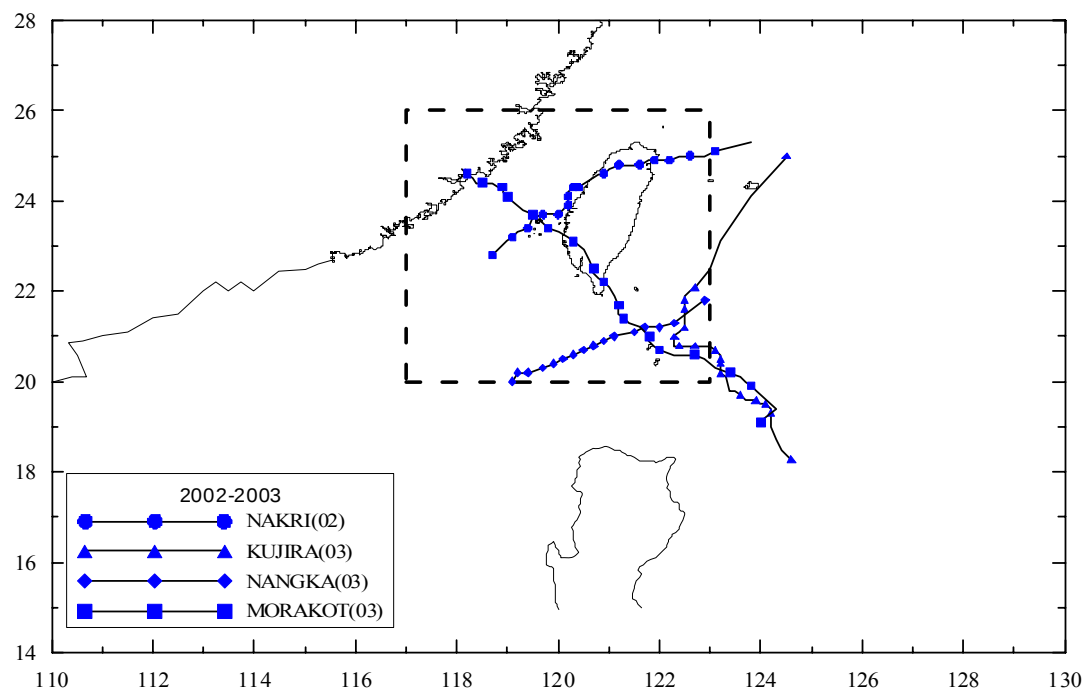
圖 3.5.2 (續 18)歷年侵臺颱風路徑圖 (2002-2003 年)
