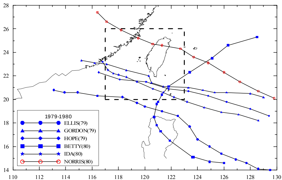
圖 3.5.2 (續 4) 歷年侵臺颱風路徑圖 (1979-1980 年)
