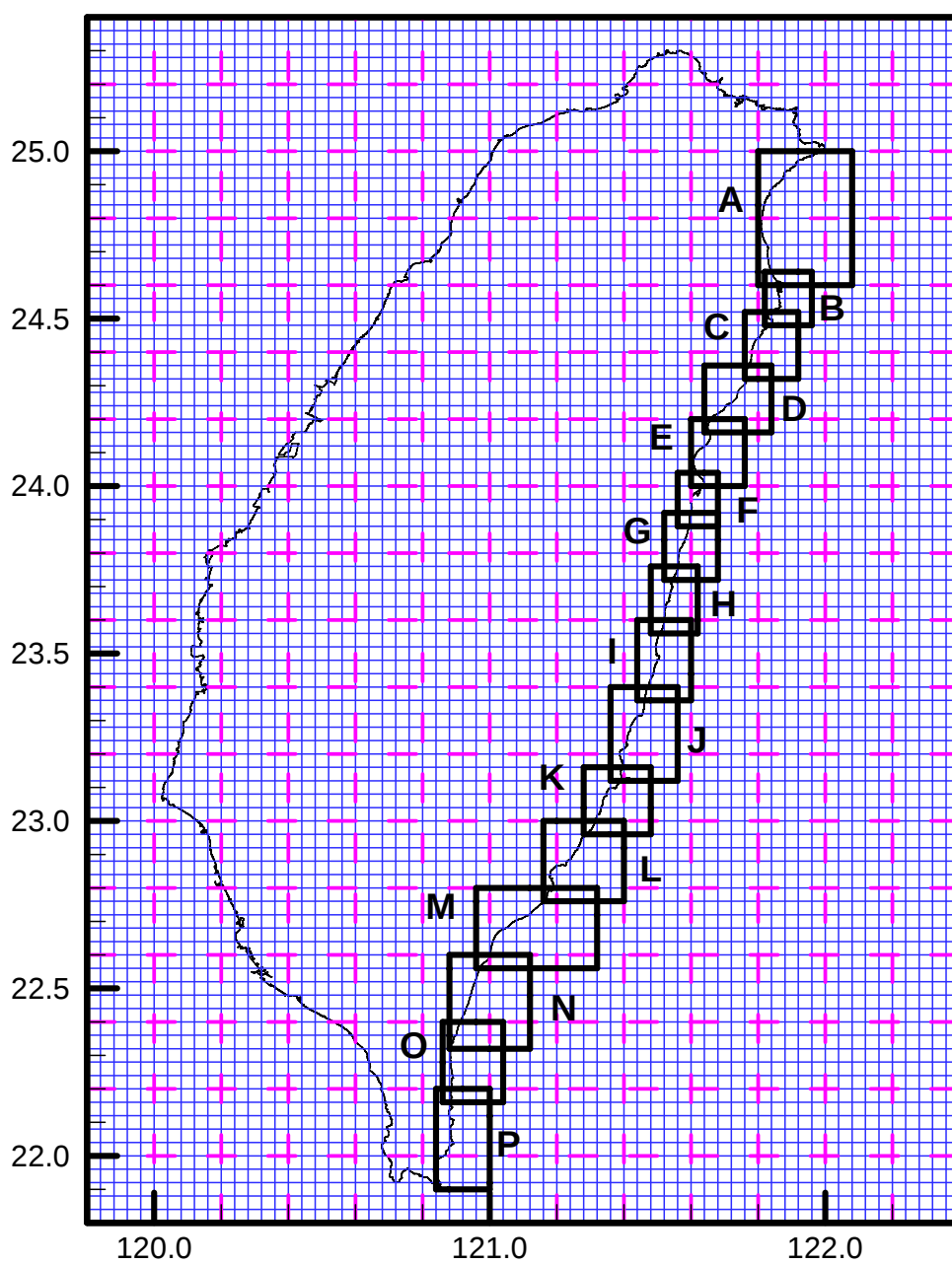
圖3.2.25 近岸區域波浪模式模擬區域與全域風浪模式SWAN(細實線)及WAM(粗虛線)數值網格相關位置圖
