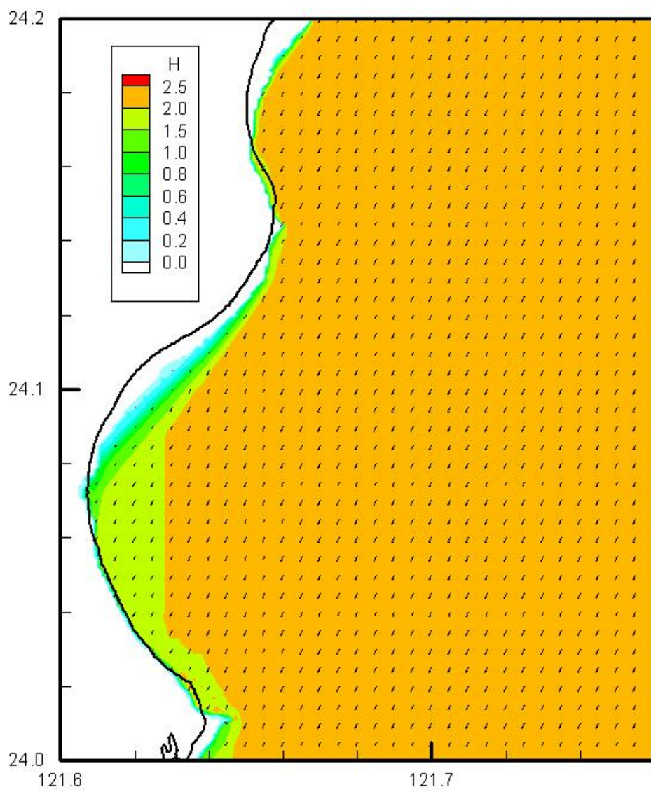
圖3.2.31 近岸區域波浪模式模擬區域E之波高及波向分佈
