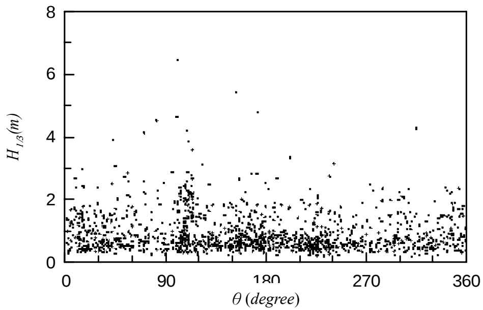
圖 3.3.20 2001 年夏季季風時期風向與示性波高關係
