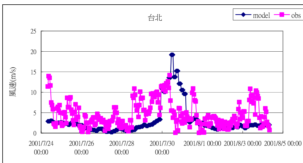
圖 2.1.10 桃芝颱風期間模式風場與臺北實測資料比對圖
