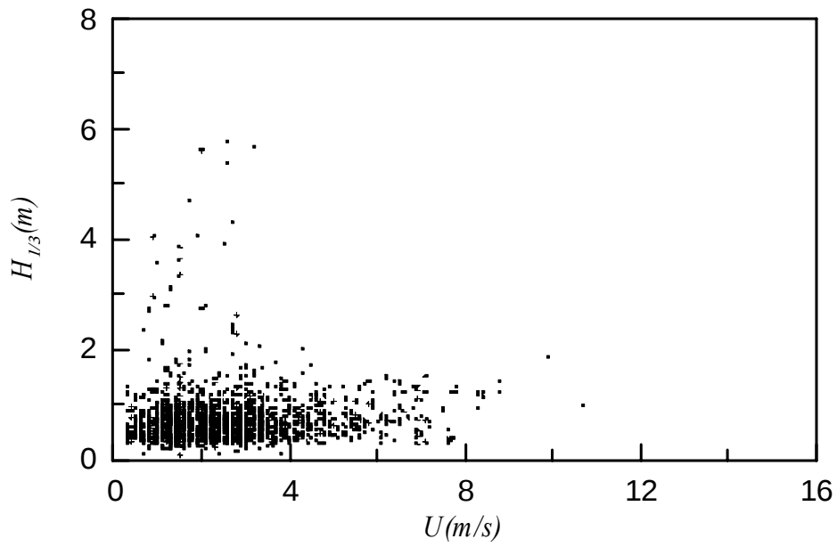
圖 3.3.17 2002 年夏季季風時期風速與示性波高關係
