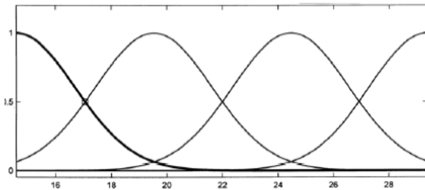
圖 3.3.23 高斯歸屬函數圖
