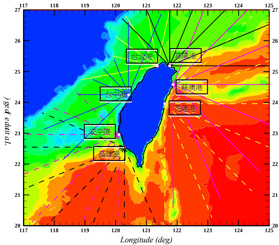
圖3.5.1 各港口推算點位置及吹風距離線示意圖
