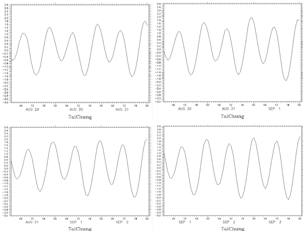
圖 6.2.18 泰利颱風期間臺中港水位預報圖（2005/08/30~09/02）
