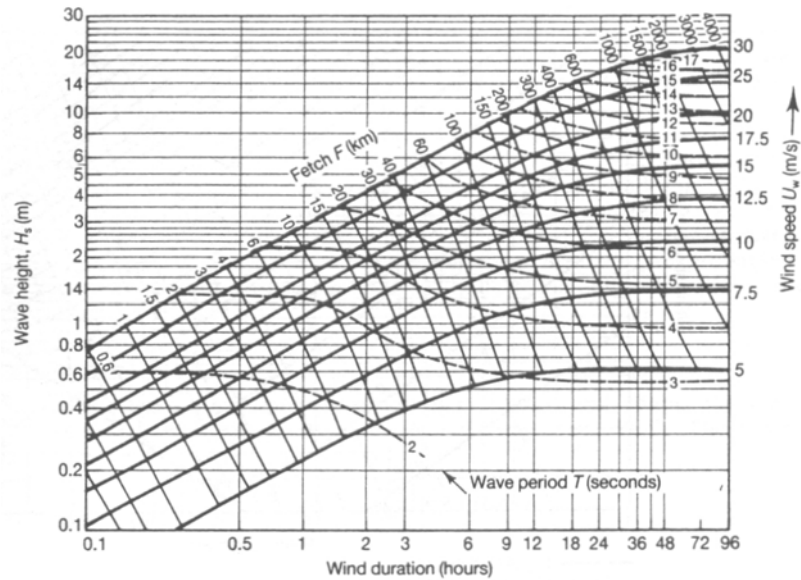
圖 3.3.12 深水波之示性波高與延時關係圖(引自 SPM,1978)
