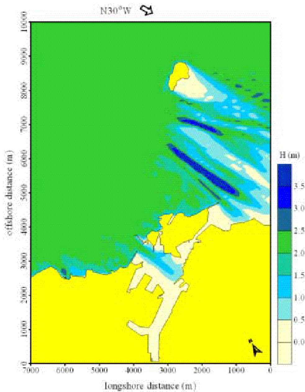
圖3.2.14 基隆港近岸波浪場EEMSE近域模式模擬結果 (奇比颱風， H=2.25\text{m} ， T=8.74\text{sec} ， S48^\circ\text{E} )
