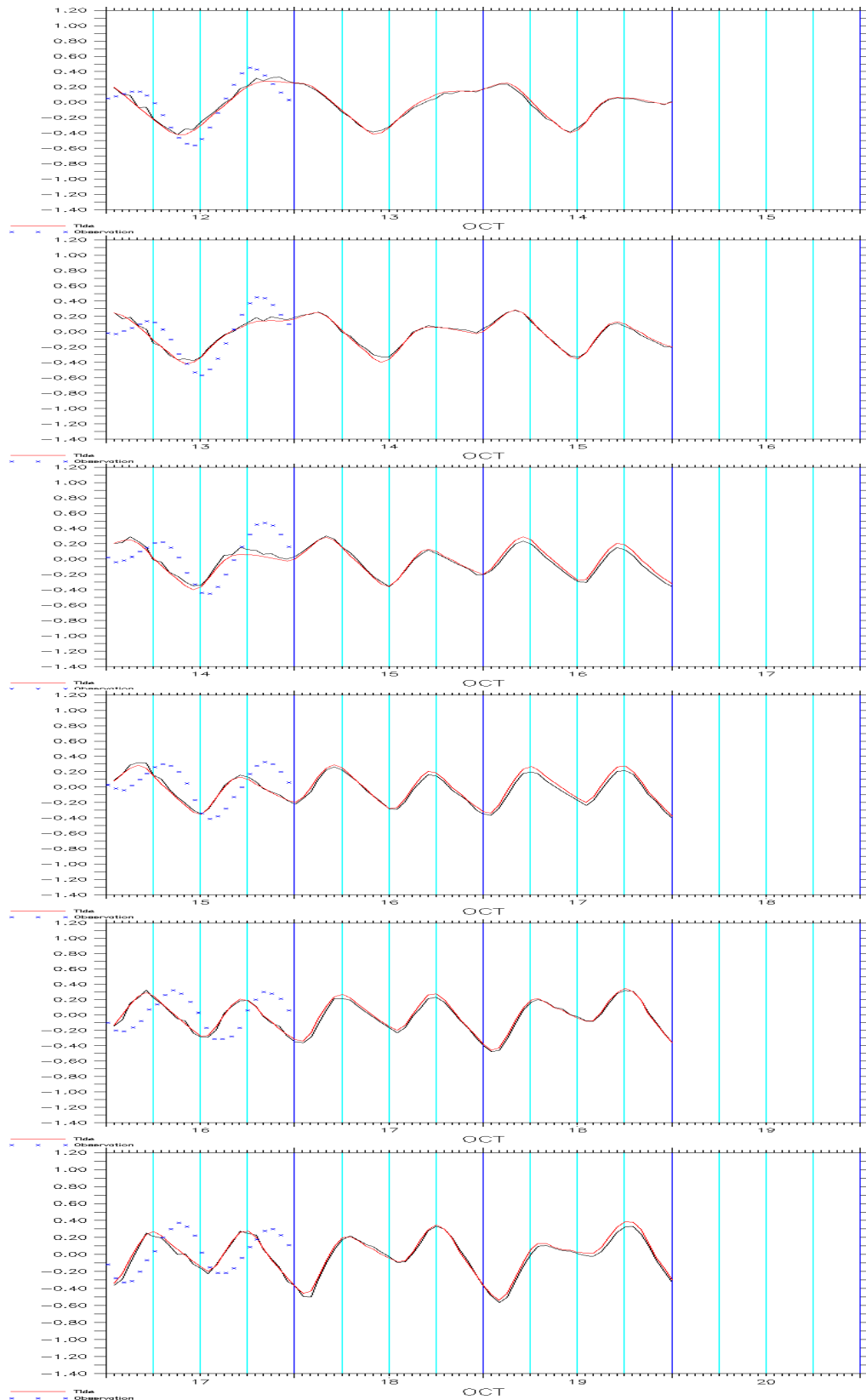
圖 6.2.29 非颱風期間基隆港水位預報圖（2005/10/13~18）
