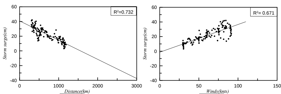
圖4.1.2.7 蘭寧颱風暴潮偏差與測站距離及中心風速相關性分析
