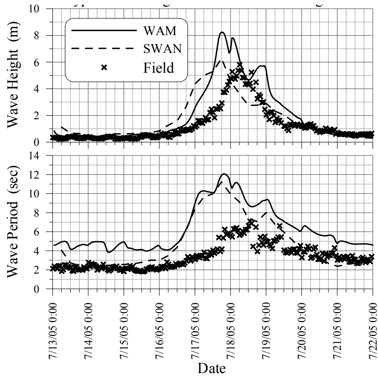
圖 3.1.7 海棠颱風侵襲時基隆港之推算波浪與觀測波浪比較圖
