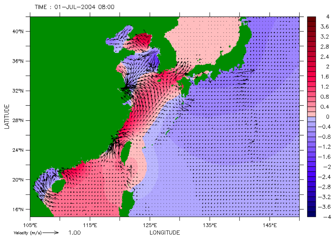
圖 4.2.1.9 敏督利颱風期間平面流場截圖
