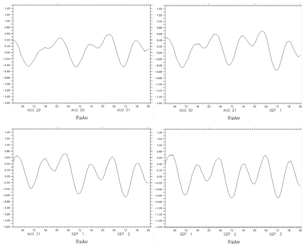
圖 6.2.17 泰利颱風期間蘇澳港水位預報圖（2005/08/30~09/02）
