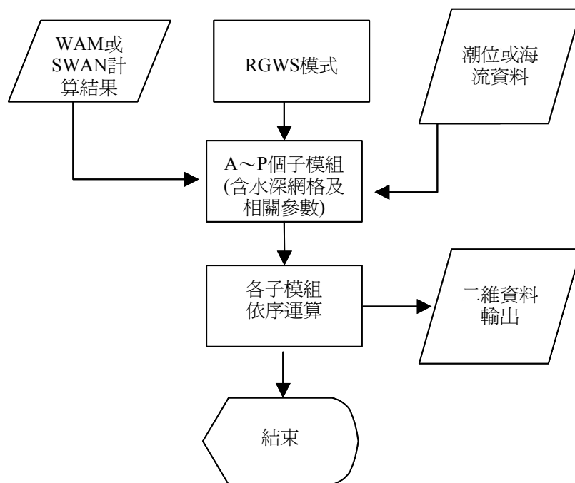
圖3.2.26 近岸區域波浪模擬系統(RGWS)計算流程
