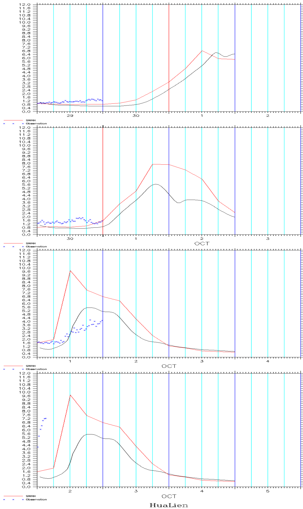
圖 6.2.24 龍王颱風期間花蓮港波高預報圖（2005/09/30~10/03）
