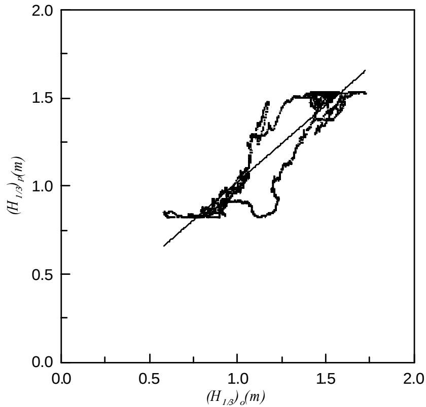
圖 3.3.30 以 2001 年之訓練輸出值與實際值的 720 小時移動平均波高之 Q-Q 圖
