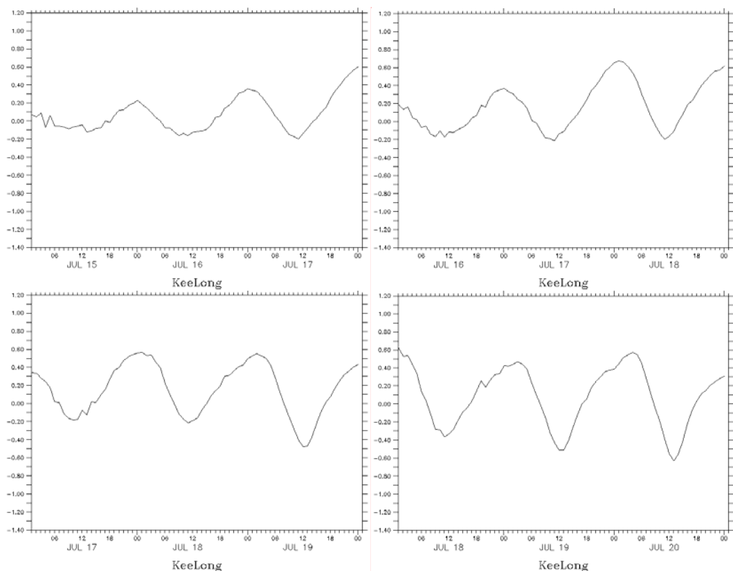
圖 6.2.8 海棠颱風期間基隆港水位預報圖（2005/07/16~07/19）
