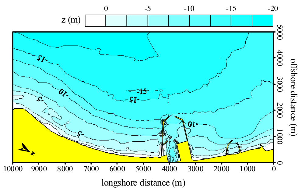
圖3.2.7 安平港近岸區域波浪模式計算範圍及水深地形分佈圖
