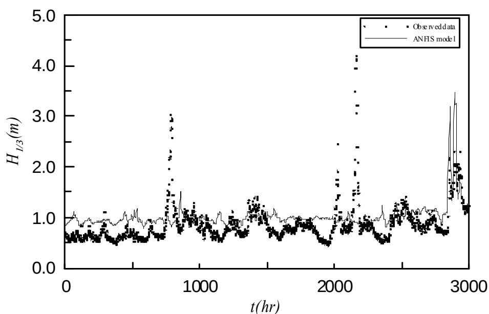
圖 3.3.43 2002 年 5~9 月實測與推算波高時序圖
