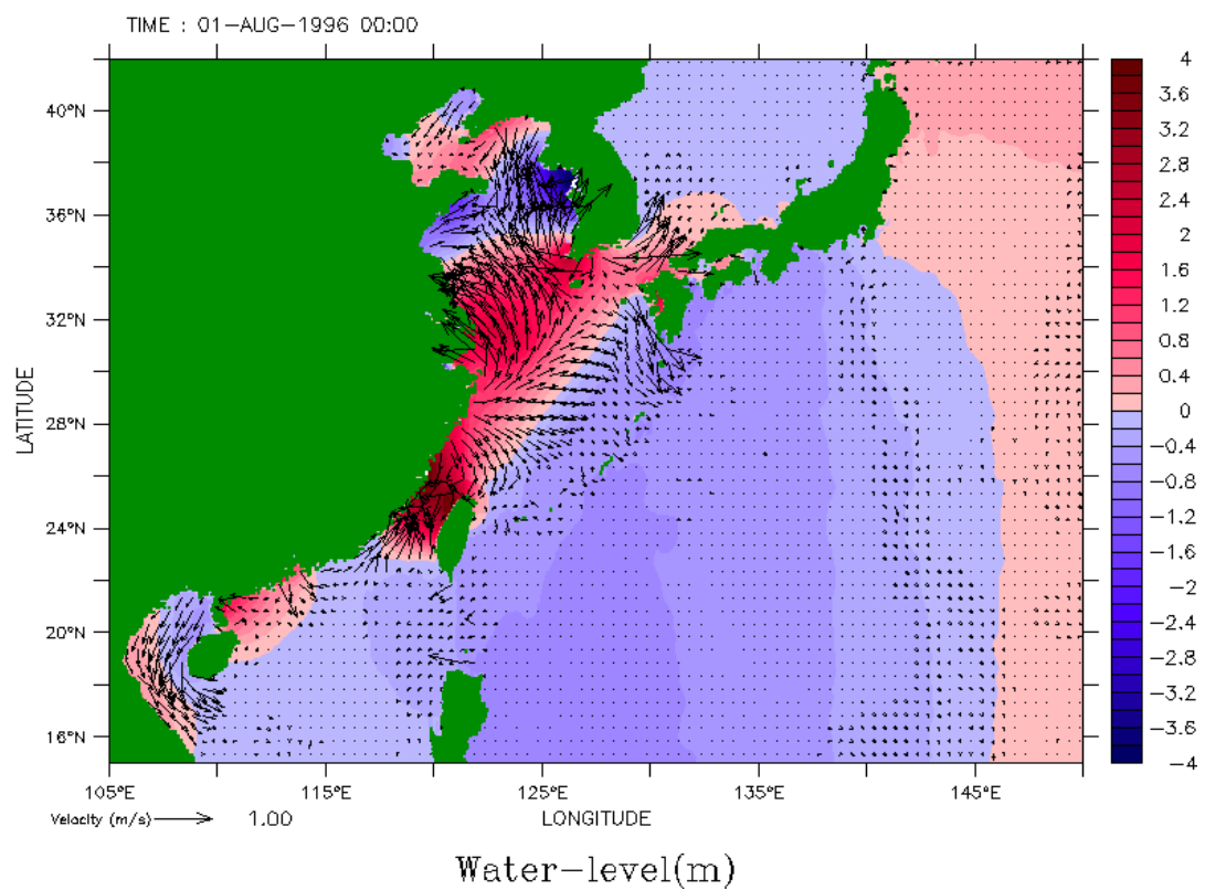
圖 4.2.1.1 賀伯颱風期間平面流場截圖
