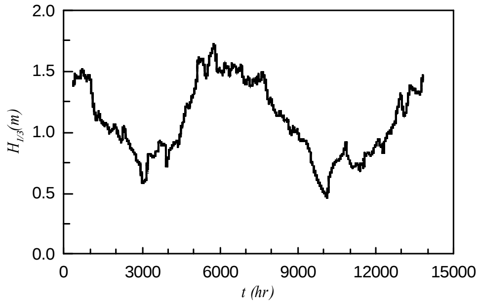
圖 3.3.27 2001-2002 花蓮站 720 小時之移動平均示性波高
