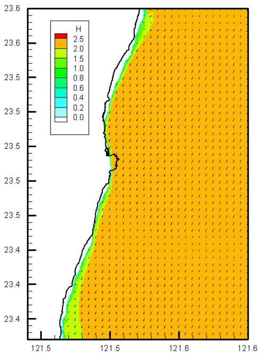
圖3.2.35 近岸區域波浪模式模擬區域I之波高及波向分佈
