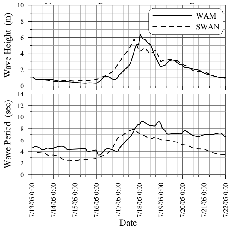
圖 3.1.11 海棠颱風侵襲時臺中港之推算波浪比較圖
