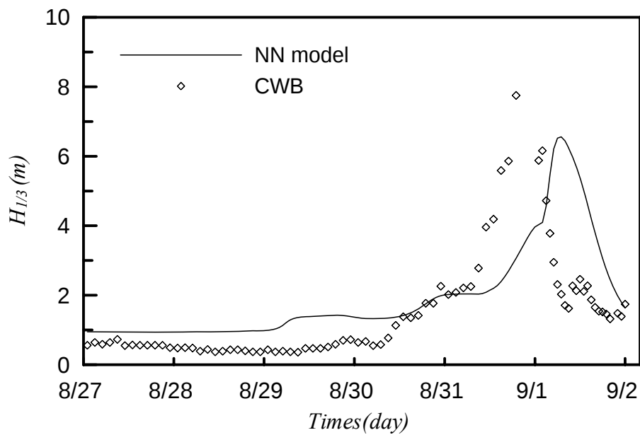
圖 3.3.11 蘇澳測站泰利颱風神經網路模式推算與實測值比較
