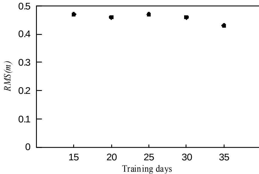
圖 3.3.33 夏季時期不同訓練時間長度所推估之示性波高 RMS 比較圖
