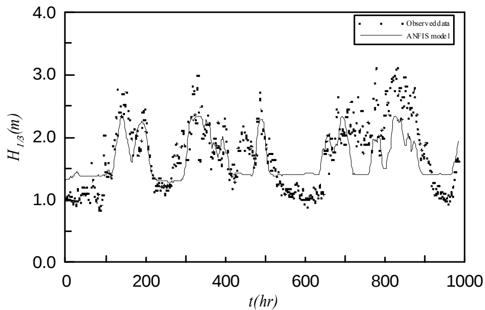
圖 3.3.41 2002 年 10-11 月實測與推算波高時序圖
