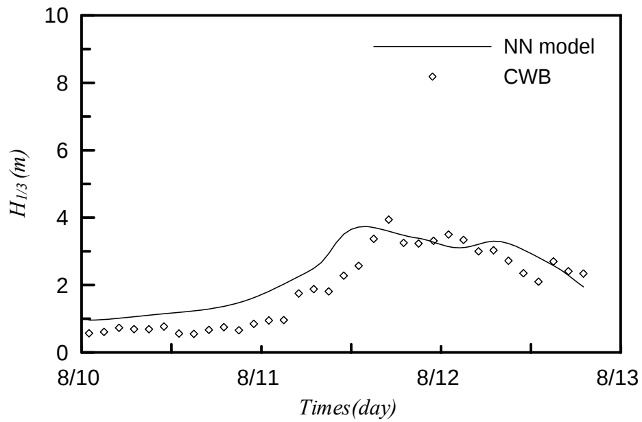
圖 3.3.9 蘇澳測站珊瑚颱風神經網路模式推算與實測值比較
