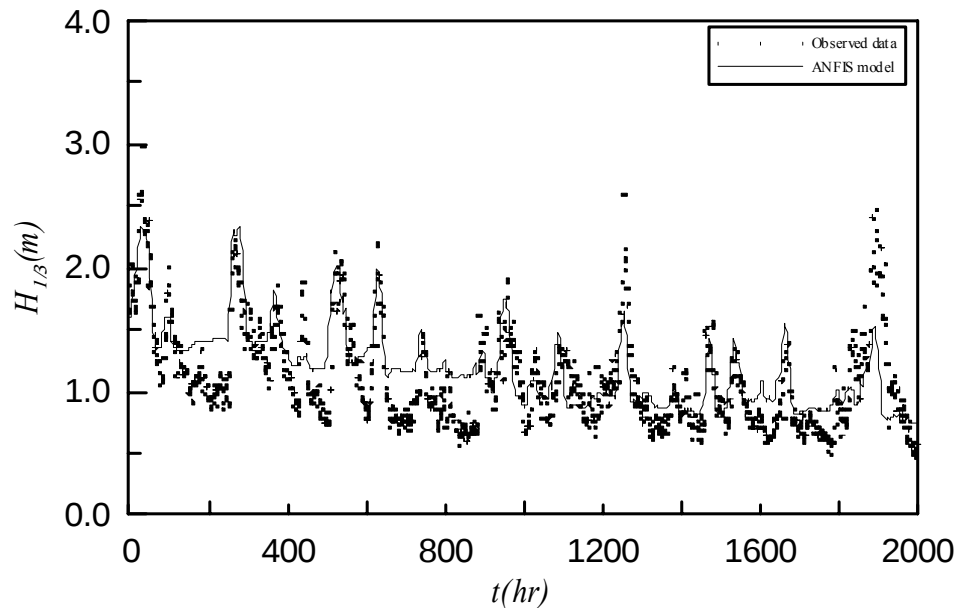
圖 3.3.38 2001 年 2-4 月實測與推算波高時序圖
