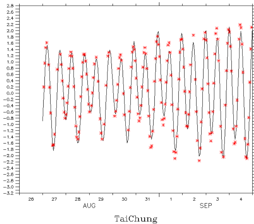
圖 4.1.1.11 泰利颱風期間臺中測站水位比對圖
