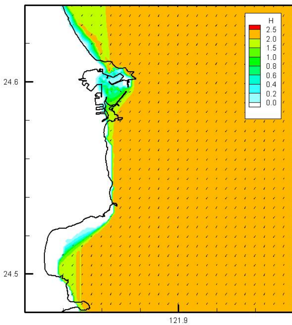
圖3.2.28 近岸區域波浪模式模擬區域B之波高及波向
