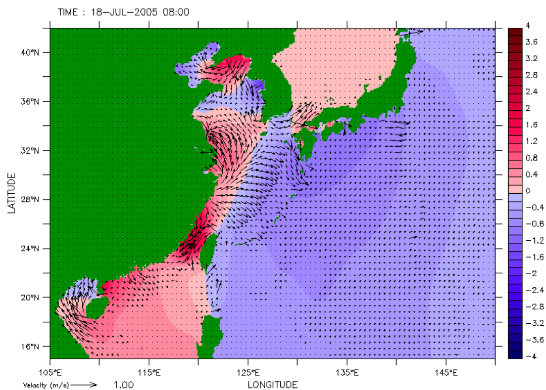
圖 4.2.1.11 海棠颱風期間平面流場截圖
