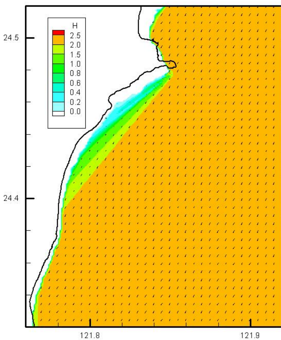
圖3.2.29 近岸區域波浪模式模擬區域C之波高及波向分佈
