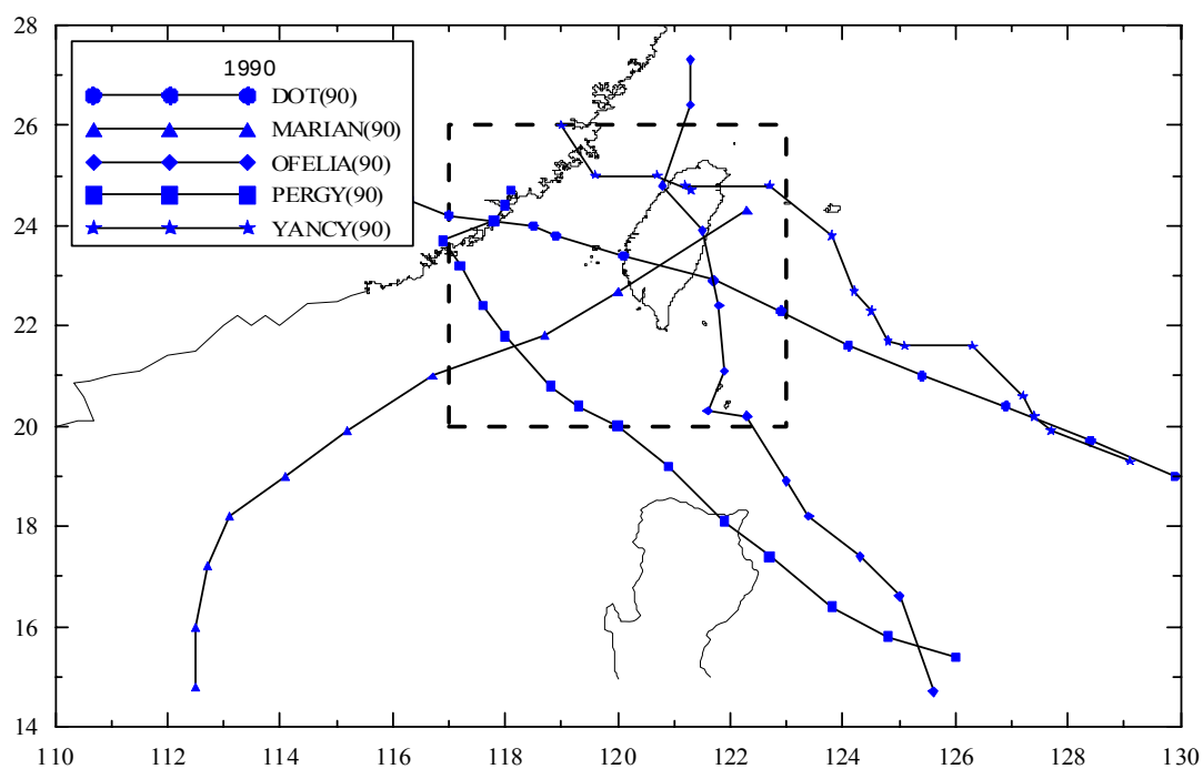
圖 3.5.2 (續 11)歷年侵臺颱風路徑圖 (1990 年)
