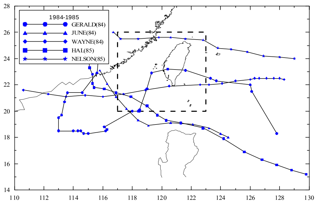
圖 3.5.2 (續 7) 歷年侵臺颱風路徑圖 (1984-1985 年)
