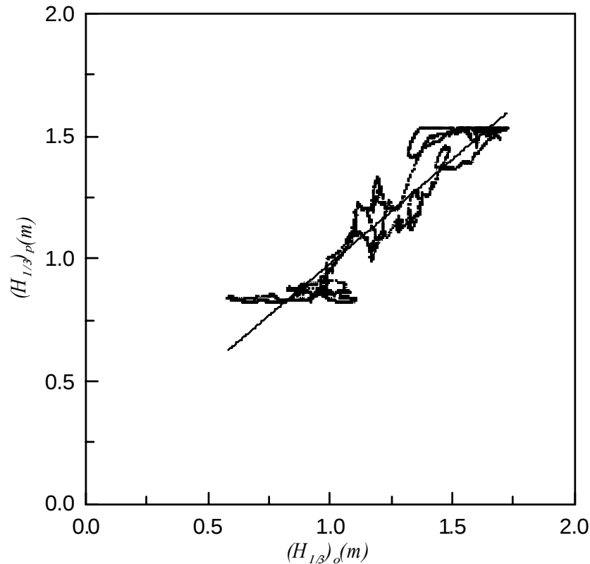
圖 3.3.27 以 2002 年之訓練輸出值與實際值的 720 小時移動平均波高之 Q-Q 圖
