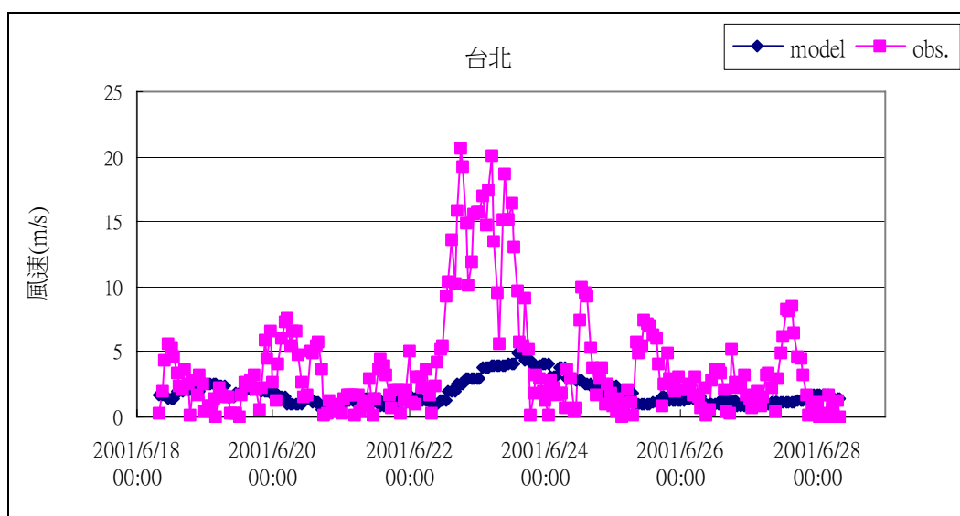
圖 2.1.12 奇比颱風期間模式風場與臺北實測資料比對圖
