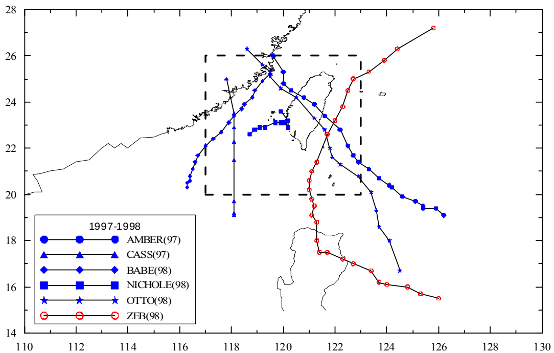
圖 3.5.2 (續 15)歷年侵臺颱風路徑圖 (1997-1998 年)
