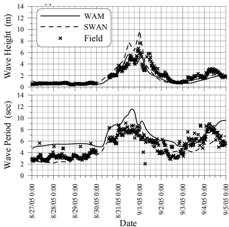
圖 3.1.16 泰利颱風侵襲時花蓮港之推算波浪與觀測波浪比較圖
