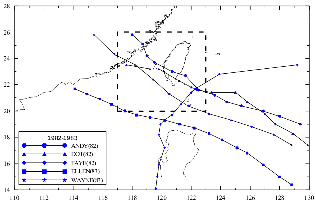
圖 3.5.2 (續 6) 歷年侵臺颱風路徑圖 (1982-1983 年)
