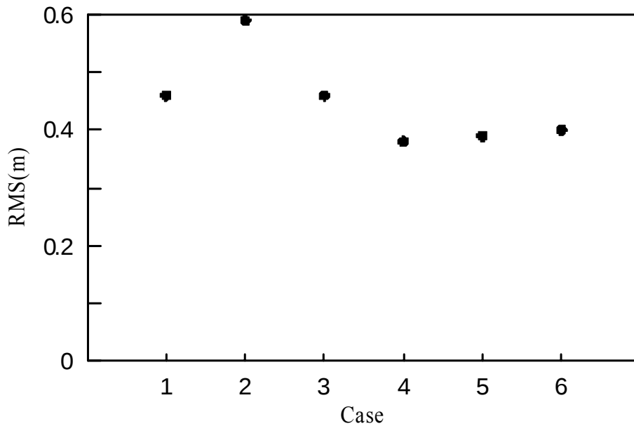
圖 3.3.37 夏季季風時期 Case1- Case6 推估波高之 RMS 比較圖
