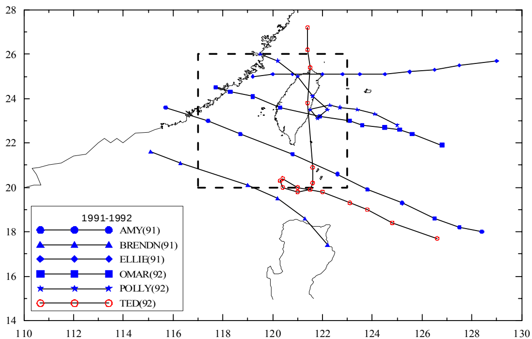
圖 3.5.2 (續 12)歷年侵臺颱風路徑圖 (1991-1992 年)
