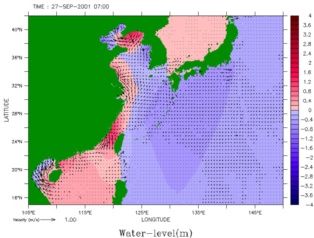
圖 4.2.1.6 利奇馬颱風期間平面流場截圖
