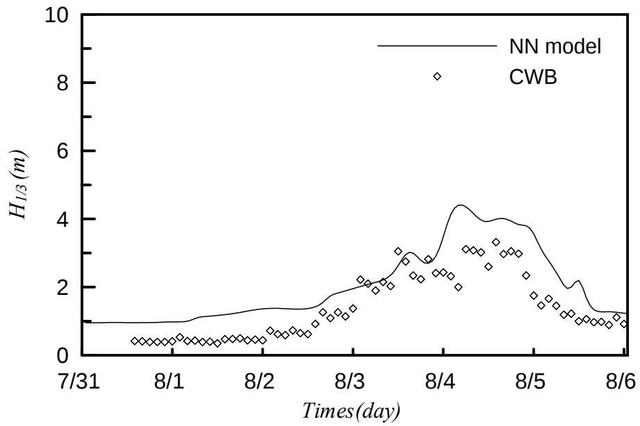
圖 3.3.6 花蓮測站馬莎颱風神經網路模式推算與實測值比較
