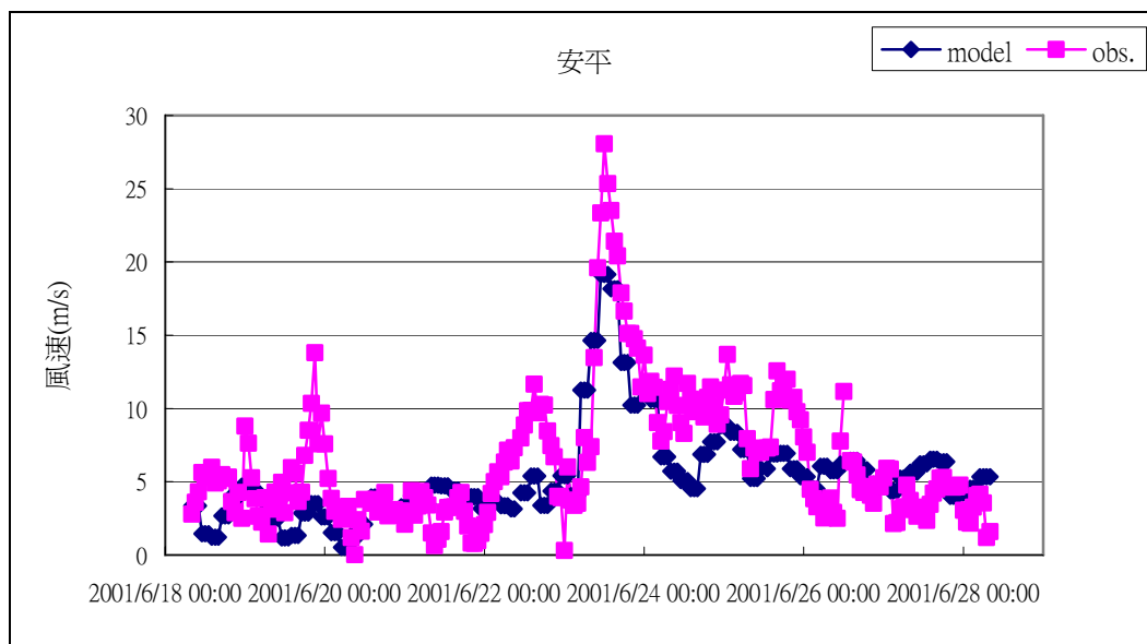
圖 2.1.11 奇比颱風期間模式風場與安平實測資料比對圖
