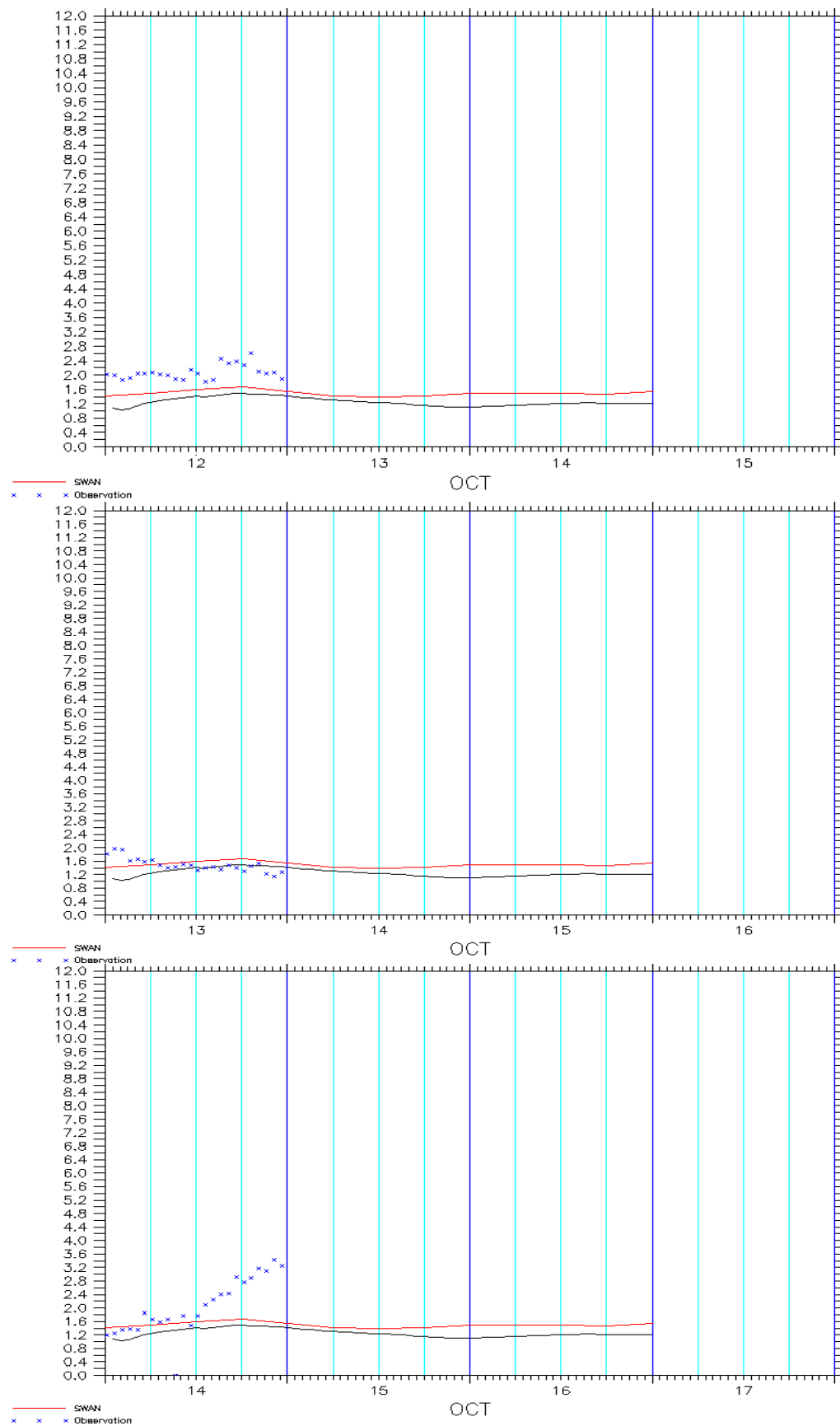
圖 6.2.33 非颱風期間基隆港波高預報圖 (2005/10/13~15)
