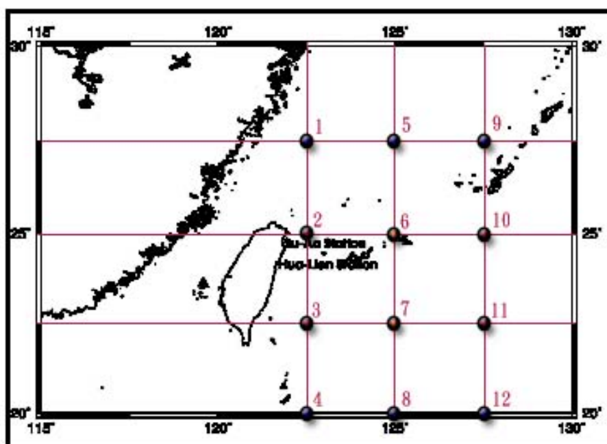
圖 3.3.2 12 個虛擬觀測站位置
