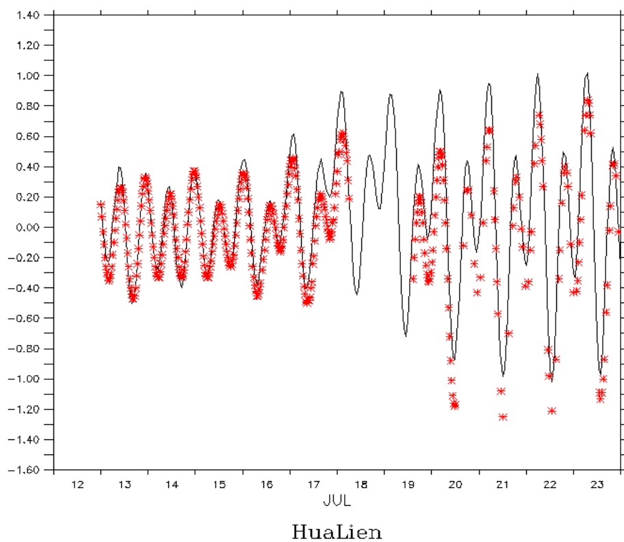
圖 4.1.1.6 海棠颱風期間花蓮測站水位比對圖
