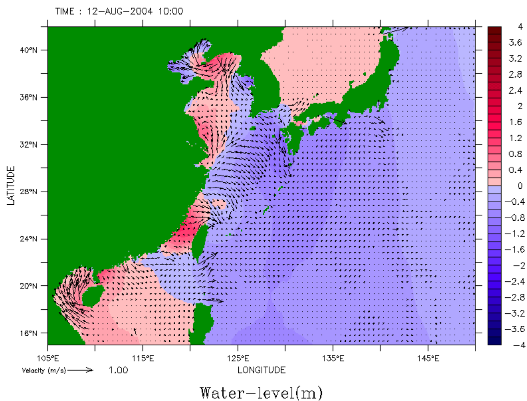
圖 4.2.1.10 蘭寧颱風期間平面流場截圖
