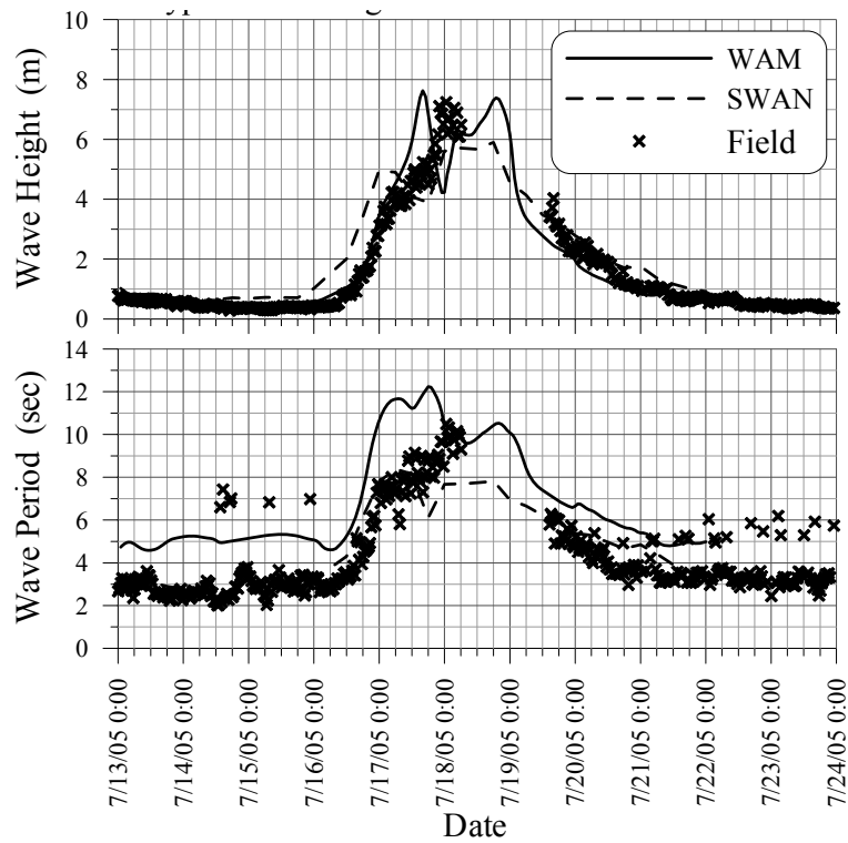
圖 3.1.9 海棠颱風侵襲時花蓮港之推算波浪與觀測波浪比較圖
