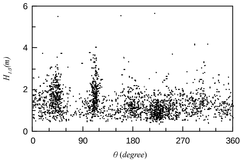
圖 3.3.18 2001 年冬季季風時期風向與示性波高關係
