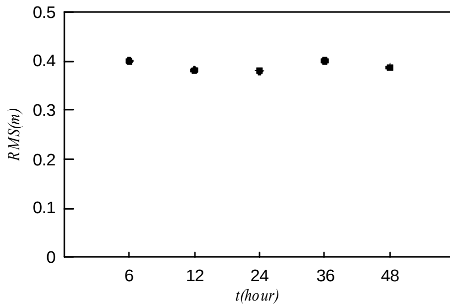
圖 3.3.35 夏季時期不同時間以移動平均風速推估之示性波高 RMS 比較圖
