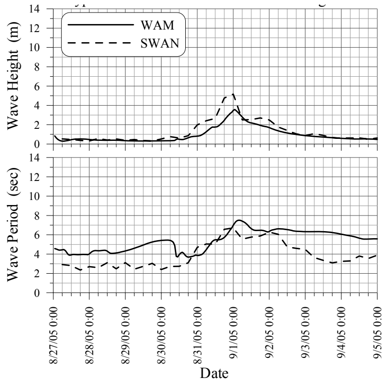
圖 3.1.17 泰利颱風侵襲時高雄港之推算波浪比較圖
