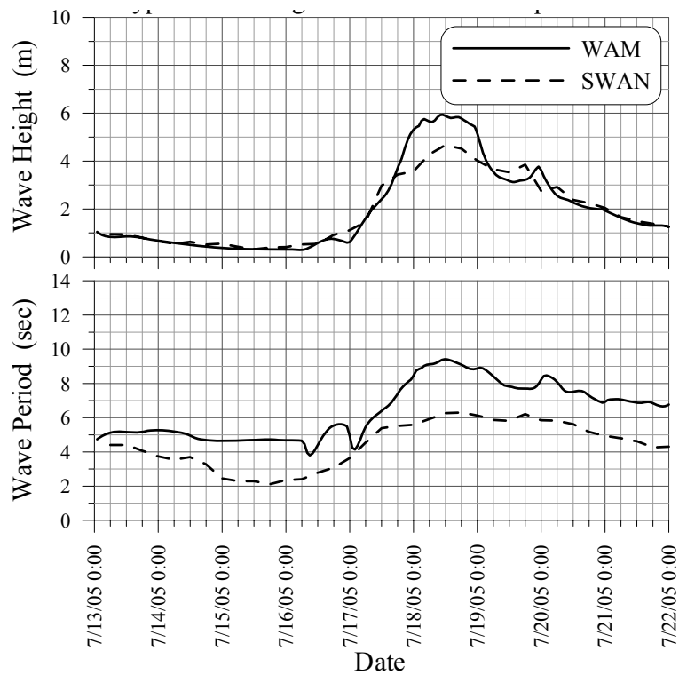
圖 3.1.12 海棠颱風侵襲時安平港之推算波浪比較圖
