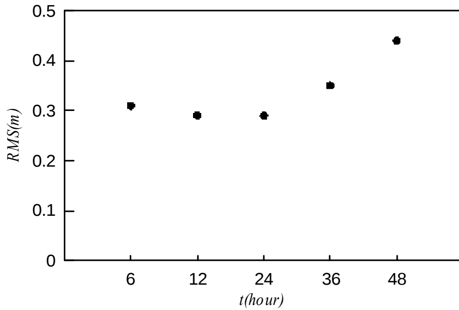
圖 3.3.34 冬季時期不同時間以移動平均風速推估之示性波高 RMS 比較圖
