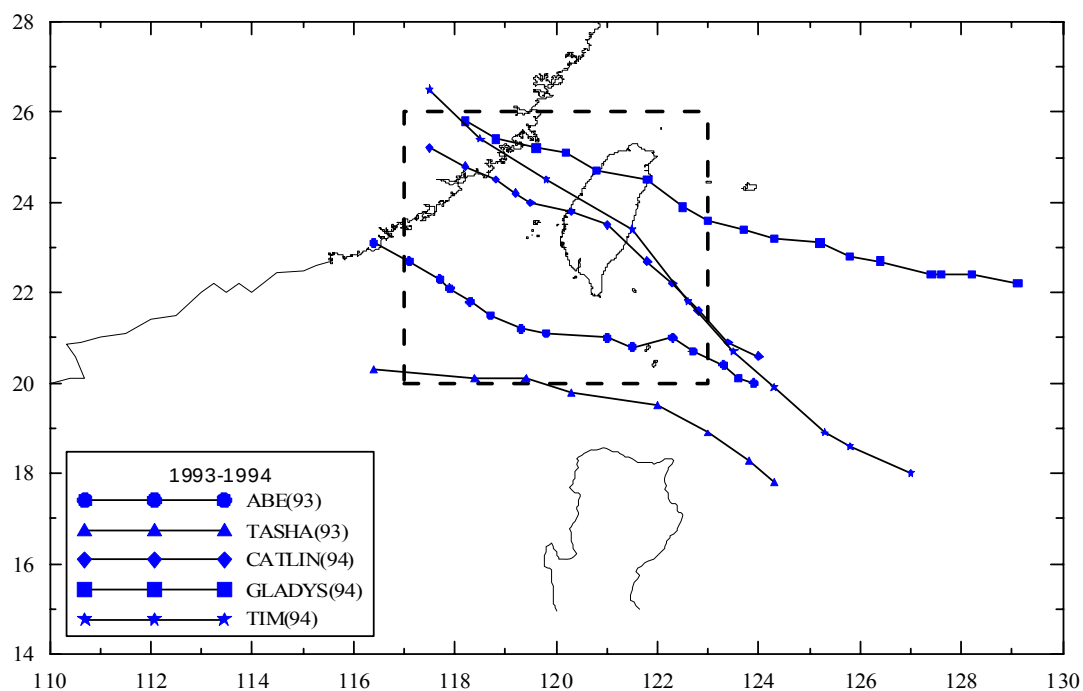
圖 3.5.2 (續 13)歷年侵臺颱風路徑圖 (1993-1994 年)
