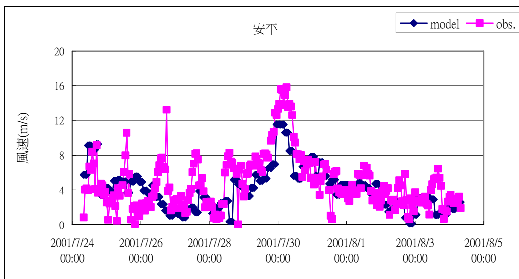
圖 2.1.9 桃芝颱風期間模式風場與安平實測資料比對圖
