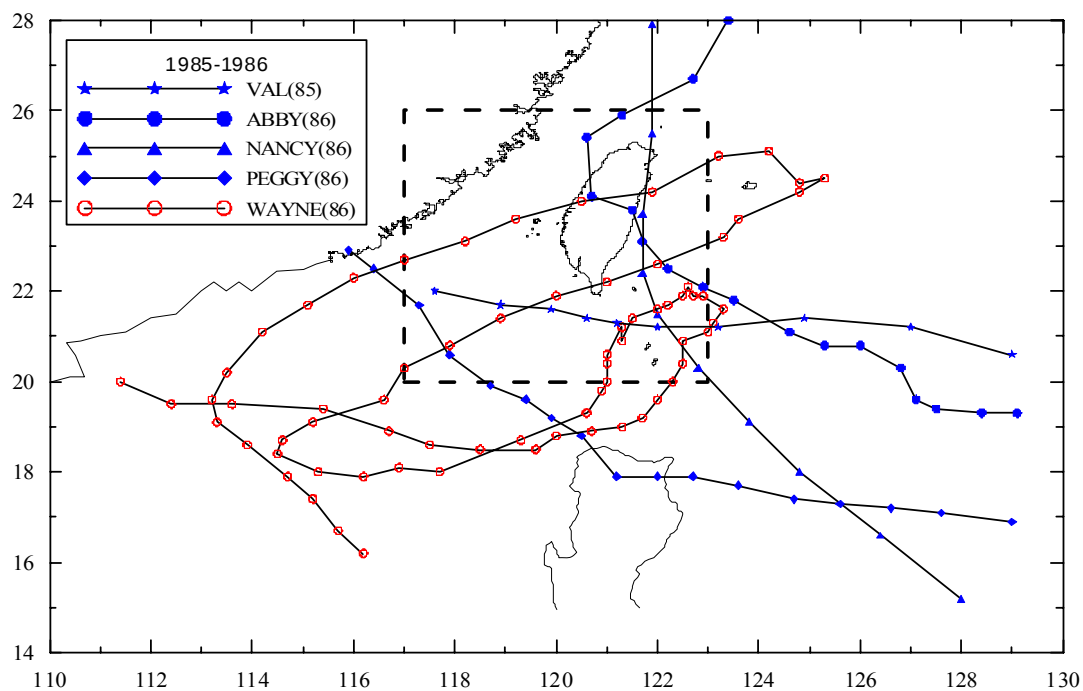
圖 3.5.2 (續 8)歷年侵臺颱風路徑圖 (1985-1986 年)
