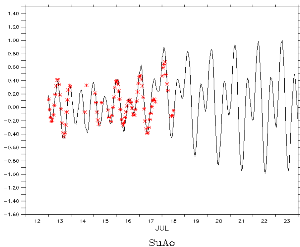
圖 4.1.1.8 海棠颱風期間蘇澳測站水位比對圖
