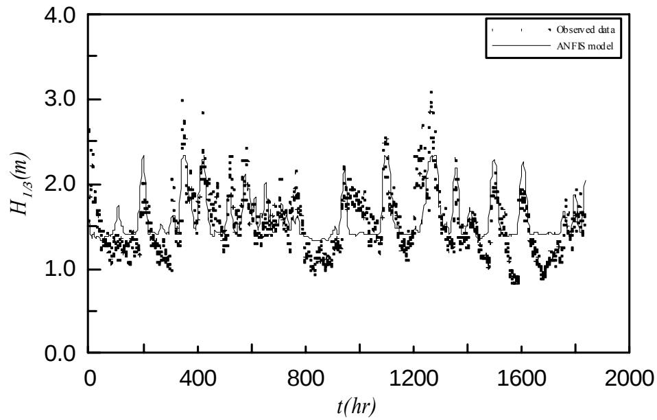
圖 3.3.40 2001 年 10-12 月實測與推算波高時序圖
