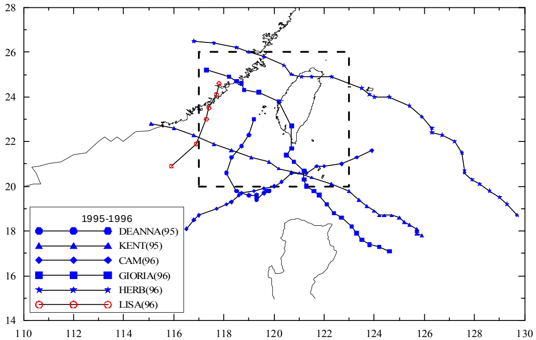
圖 3.5.2 (續 14)歷年侵臺颱風路徑圖 (1995-1996 年)
