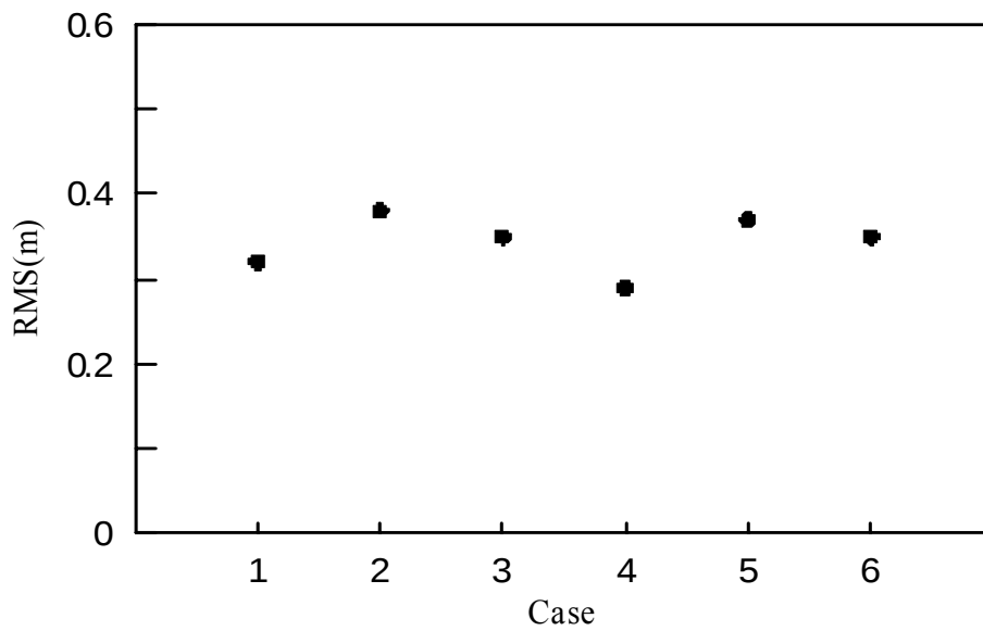
圖 3.3.36 冬季季風時期 Case1- Case6 推估波高之 RMS 比較圖
