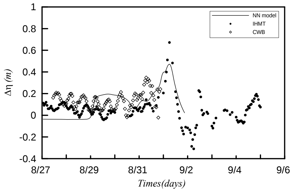
圖 4.1.2.22 泰利颱風暴潮偏差與花蓮港觀測值之比較
