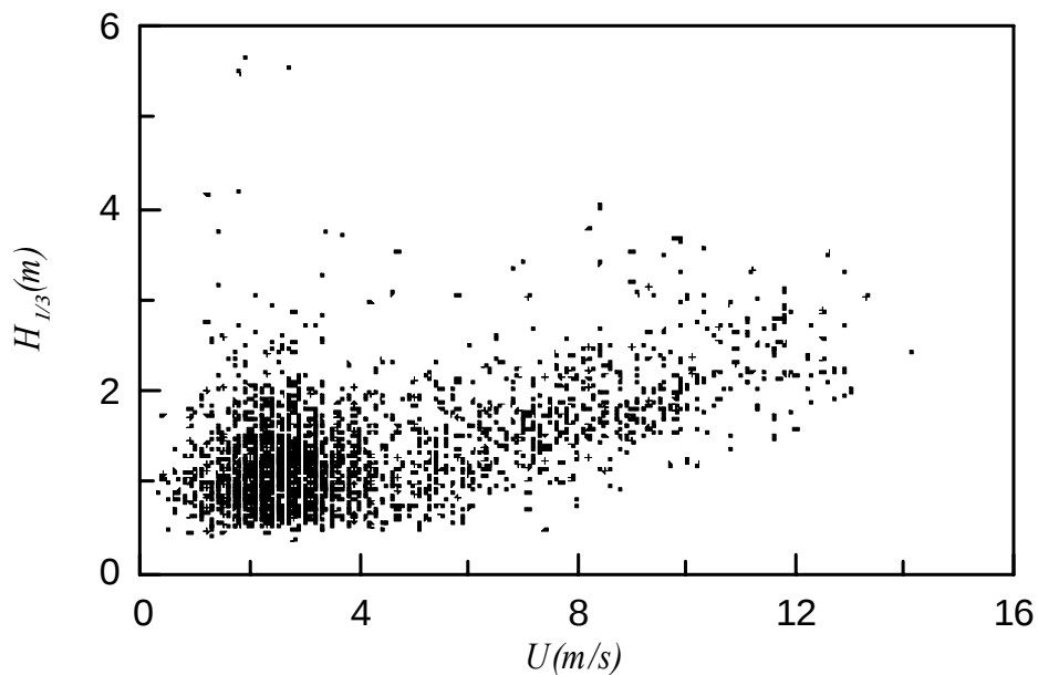
圖 3.3.14 2001 年冬季季風時期風速與示性波高關係
