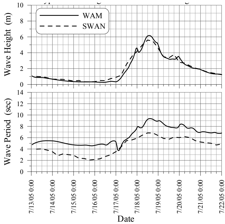
圖 3.1.13 海棠颱風侵襲時高雄港之推算波浪比較圖
