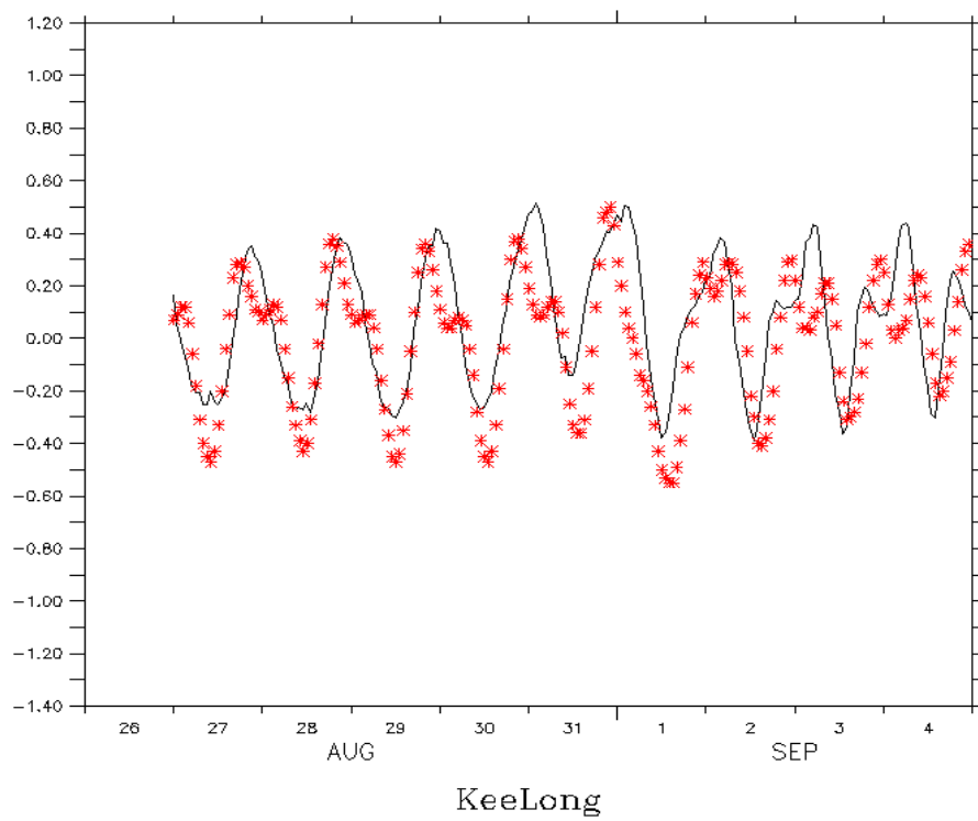
圖 4.1.1.10 泰利颱風期間基隆測站水位比對圖
