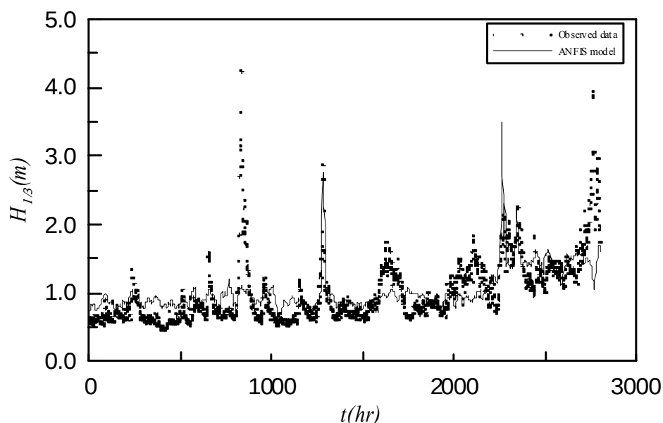
圖 3.3.42 2001 年 5-9 月實測與推算波高時序圖
