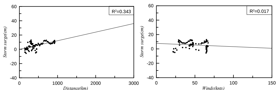
圖4.1.2.11 莫拉克颱風暴潮偏差與測站距離及中心風速相關性分析
