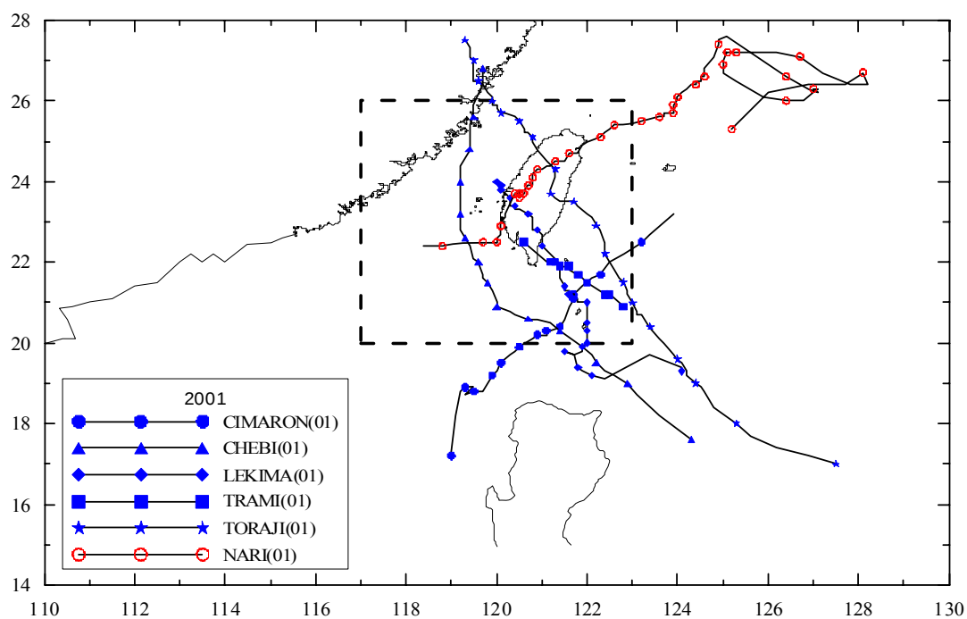
圖 3.5.2 (續 17)歷年侵臺颱風路徑圖 (2001 年)
