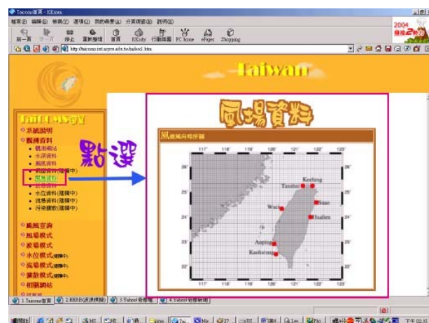
圖 5.2.24b 典型風場資料
