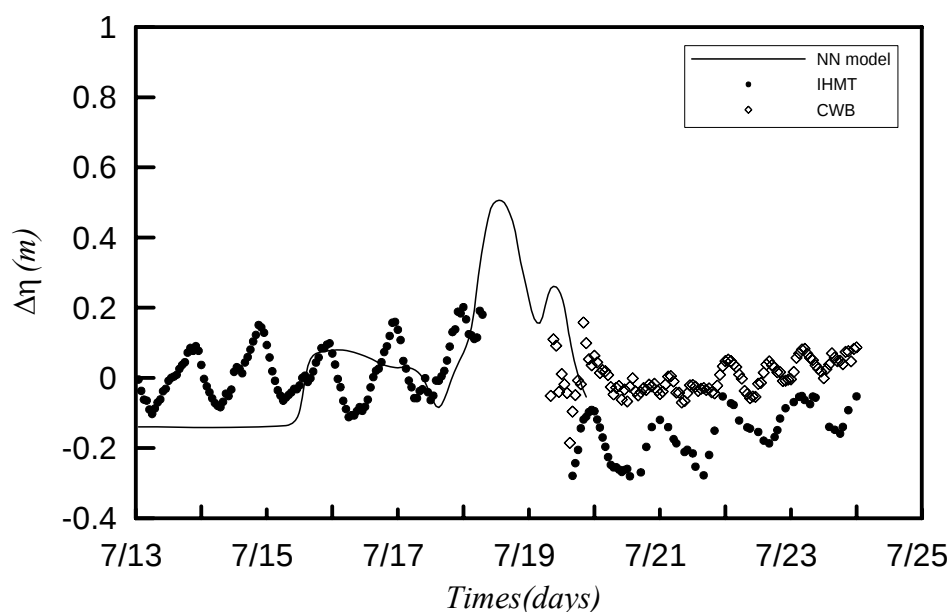
圖 4.1.2.20 海棠颱風暴潮偏差與花蓮港觀測值之比較
