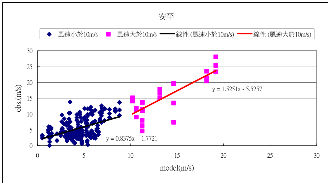
圖 2.1.15 桃芝颱風期間未修正之模式風場與安平實測資料趨勢圖
