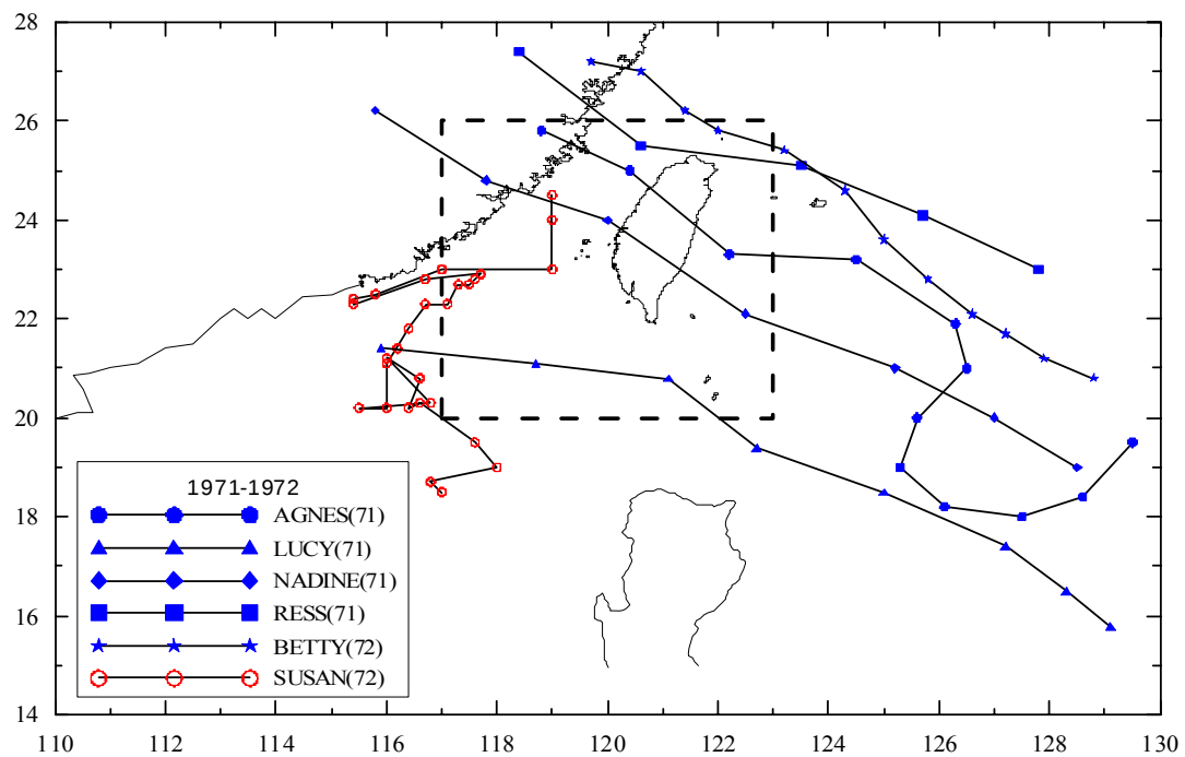
圖 3.5.2 歷年侵臺颱風路徑圖 (1971-1972 年)
