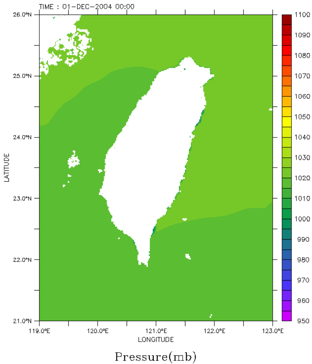
圖 2.3.3 中央氣象局 NFS 風壓模式臺灣海域(5KM)等氣壓圖
