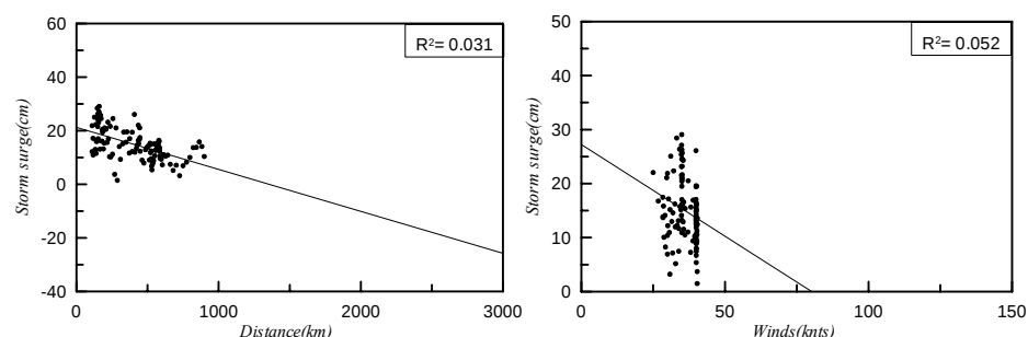
圖4.1.2.10 娜克莉颱風暴潮偏差與測站距離及中心風速相關性分析
