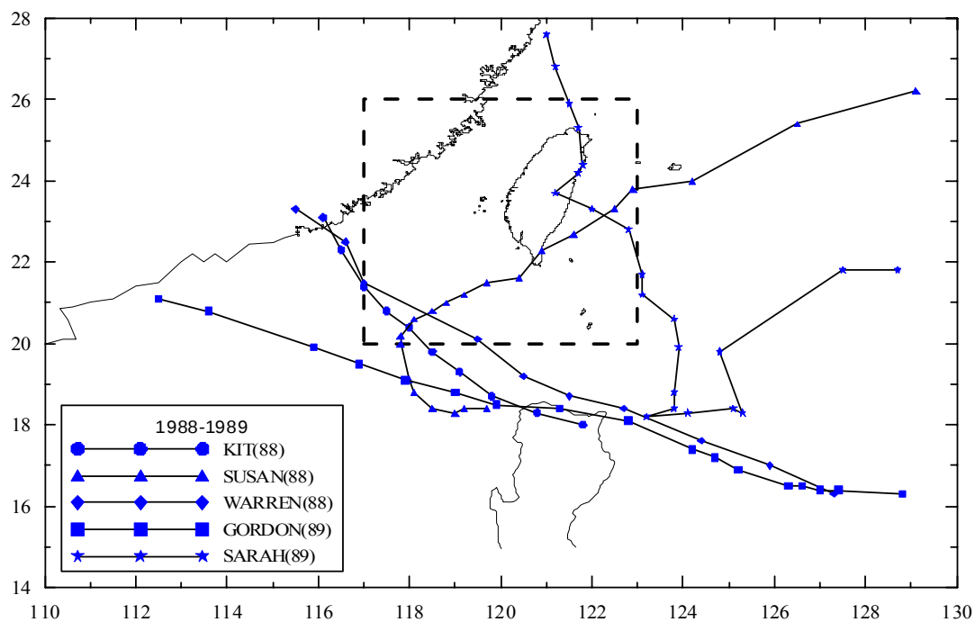
圖 3.5.2 (續 10)歷年侵臺颱風路徑圖 (1988-1989 年)
