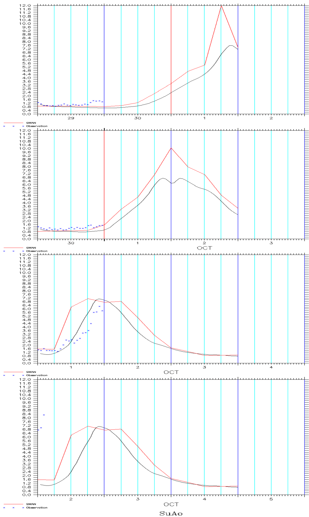
圖 6.2.26 龍王颱風期間蘇澳港波高預報圖（2005/09/30~10/03）
