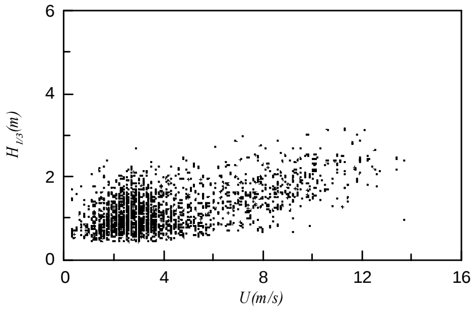
圖 3.3.15 2002 年冬季季風時期風速與示性波高關係
