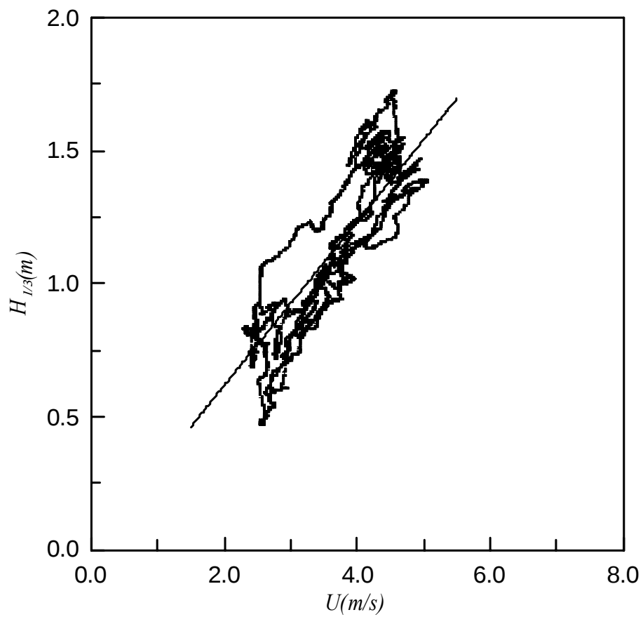
圖 3.3.28 2001-2002 花蓮站 720 小時之移動平均風速與 720 小時之移動平均示性波高 Q-Q 圖
