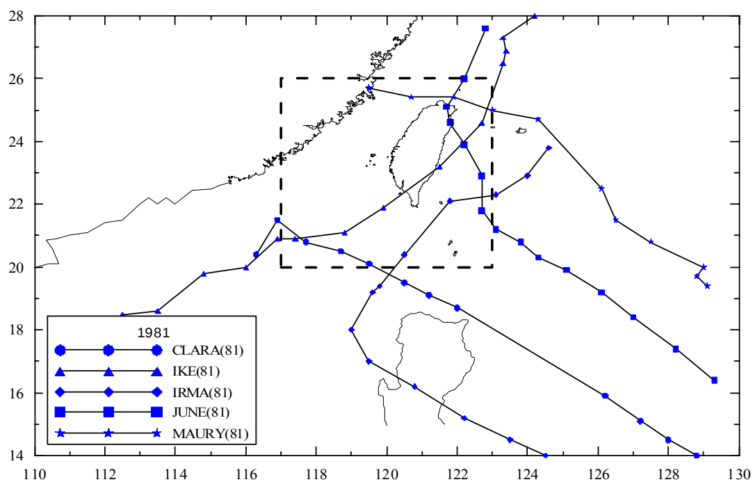
圖 3.5.2 (續 5) 歷年侵臺颱風路徑圖 (1981 年)
