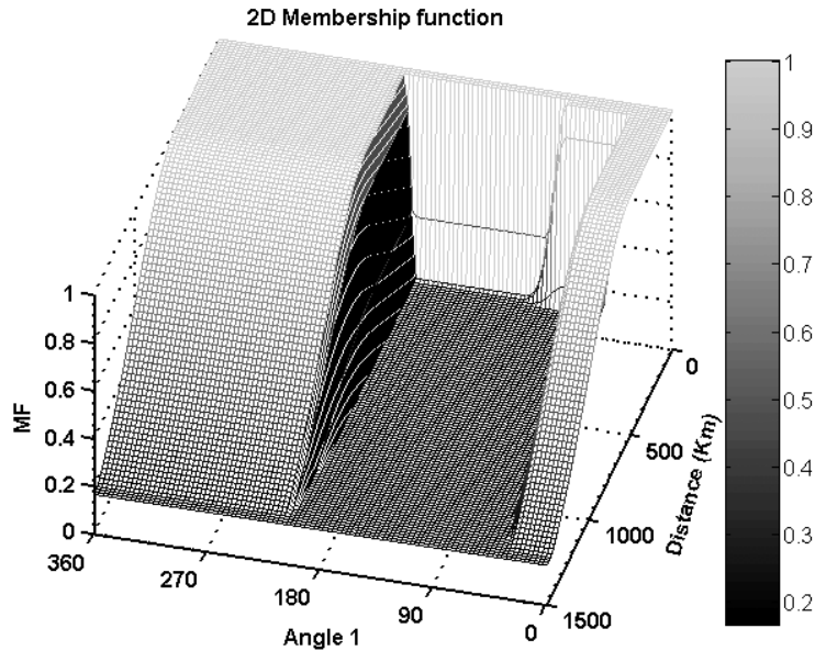
圖 4.1.2.15 陸地效應二維模糊關係函數
