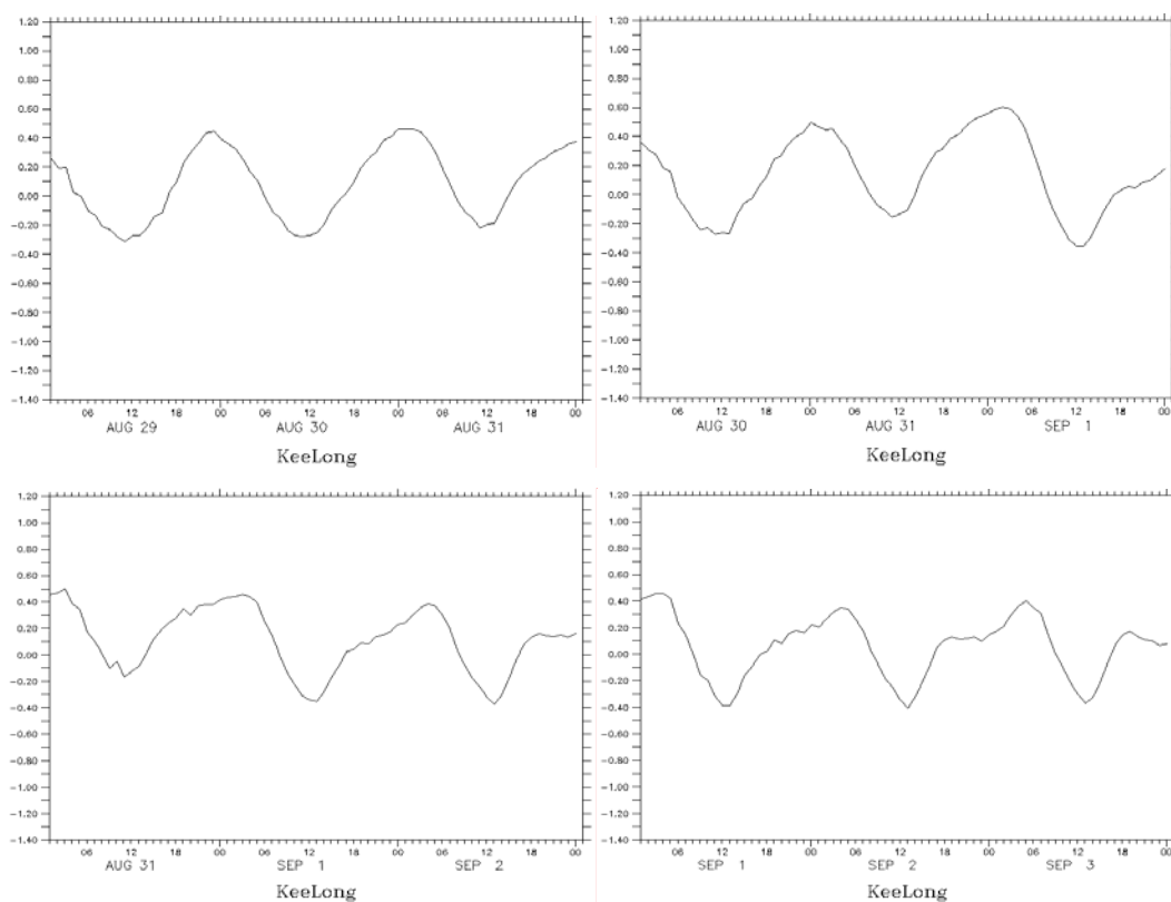
圖 6.2.16 泰利颱風期間基隆港水位預報圖（2005/08/30~09/02）
