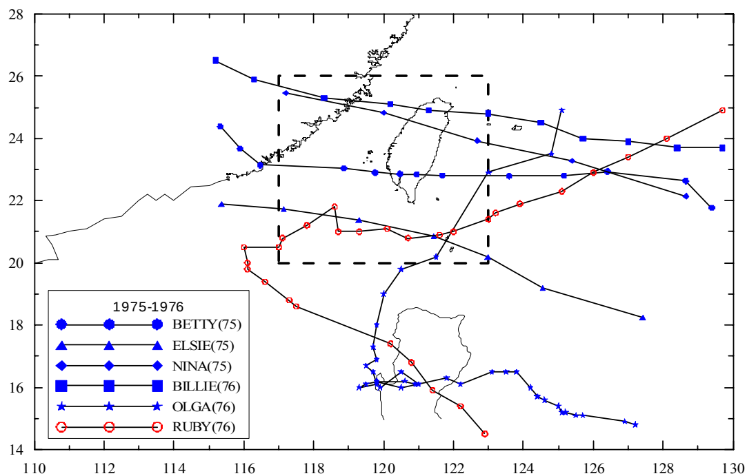
圖 3.5.2 (續 2) 歷年侵臺颱風路徑圖 (1975-1976 年)
