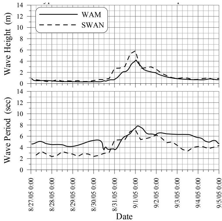
圖 3.1.19 泰利颱風侵襲時安平港之推算波浪比較圖
