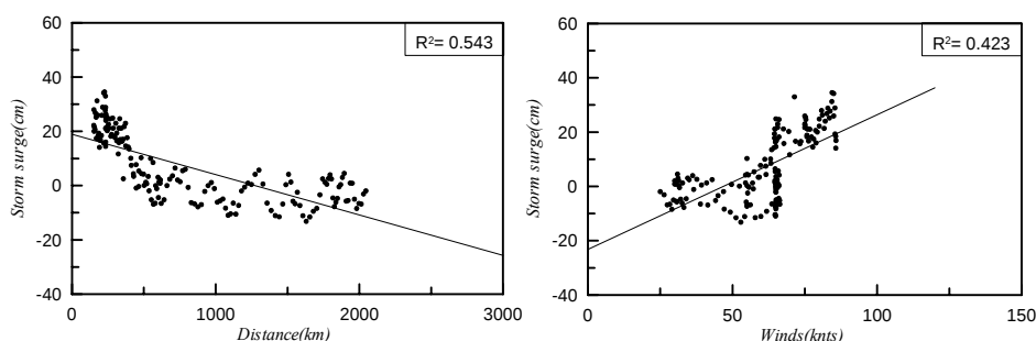
圖4.1.2.8 艾利颱風暴潮偏差與測站距離及中心風速相關性分析
