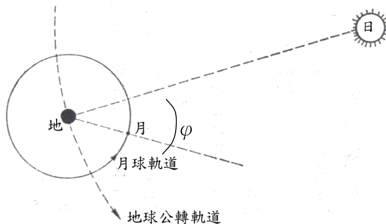
圖 4.1.2.1 太陽、月球相對地球角度
