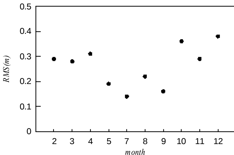
圖 3.3.44 2001 年各月份之推估波高 RMS 值
