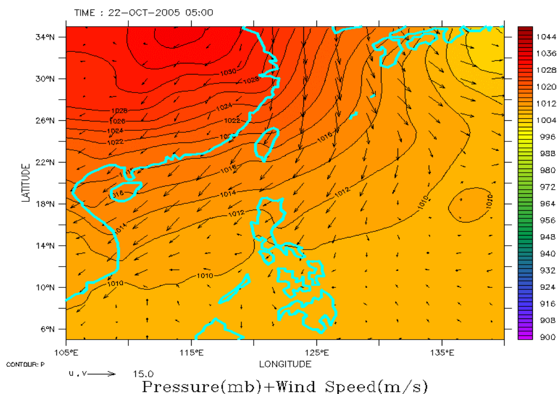
圖 4.1.1.5 氣象局之動態風場氣壓場 (根據中央氣象局預報資料繪製)
