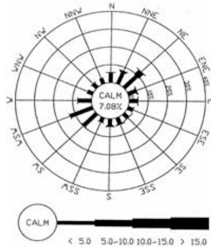
圖 3.3.13 花蓮港年平均風力統計分布(資料來源：港研所，1996)
