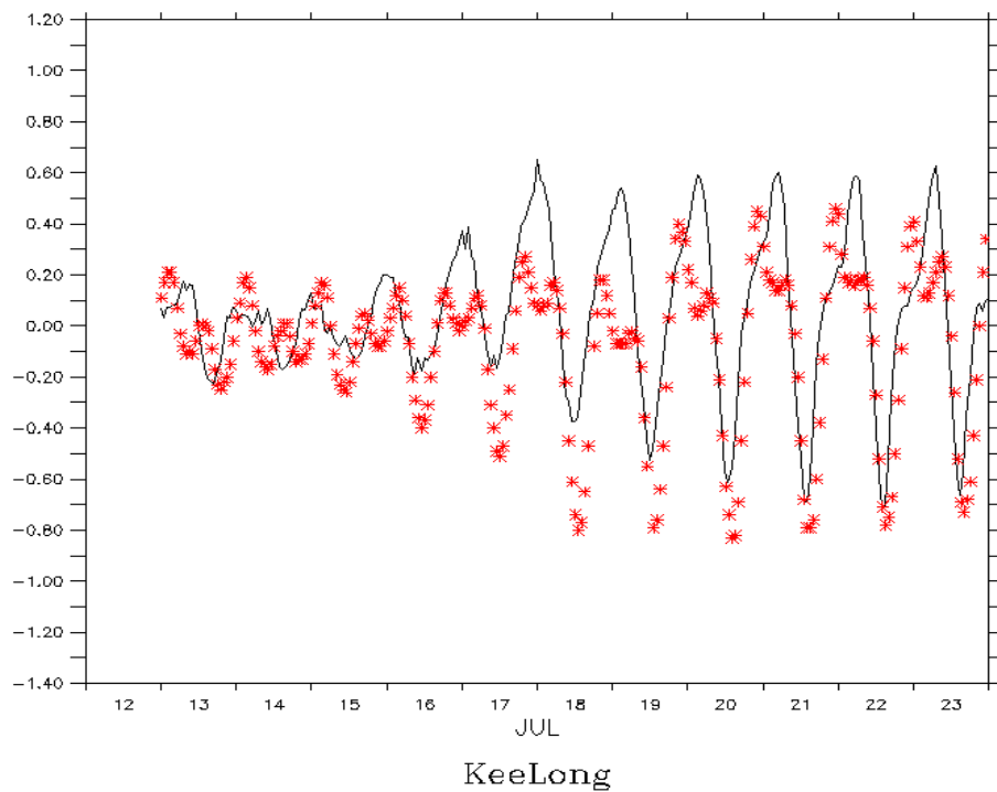
圖 4.1.1.7 海棠颱風期間基隆測站水位比對圖
