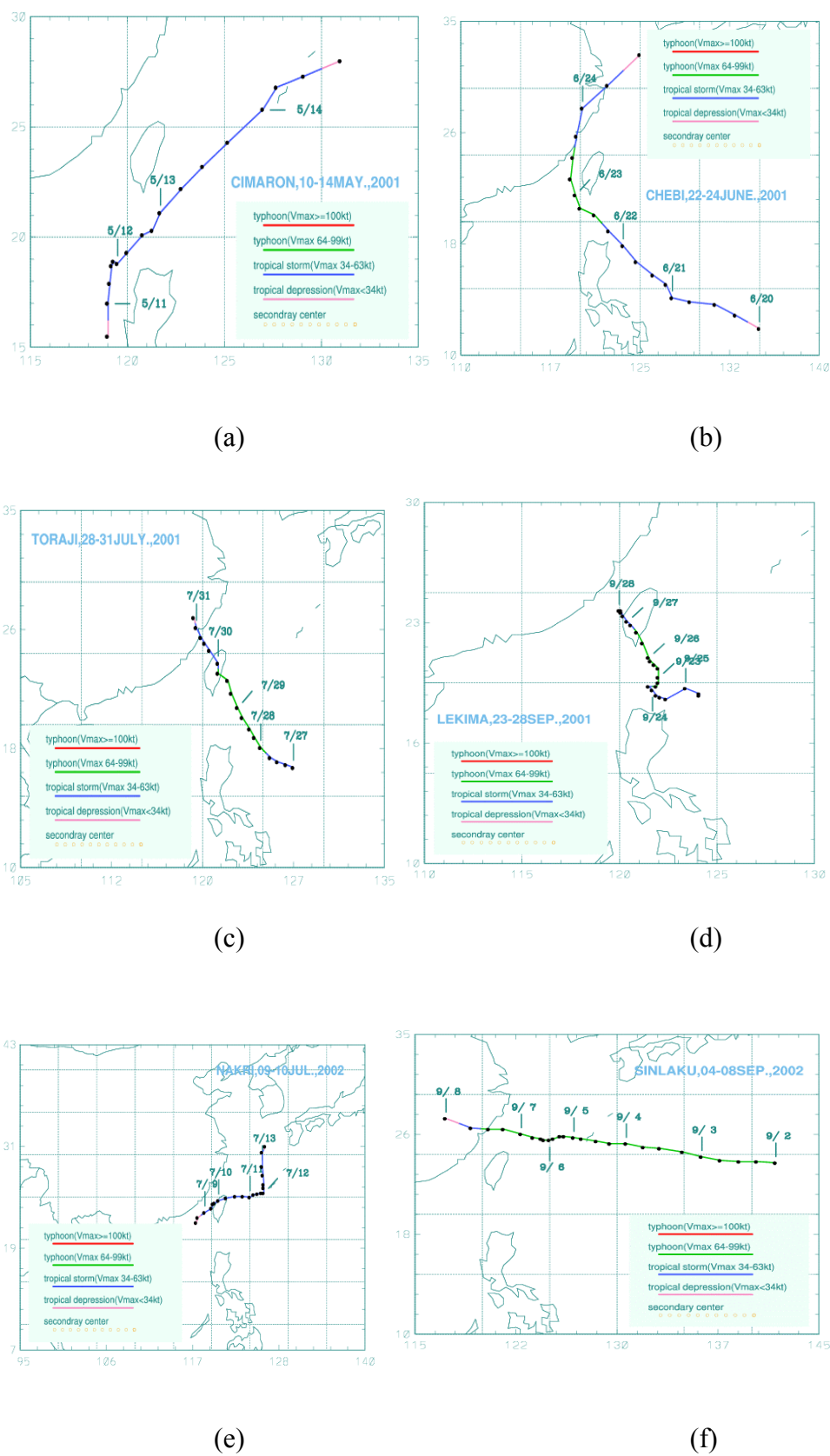
圖 2.1.1 六個颱風路徑圖(a)西馬隆(b)奇比(c)桃芝(d)利奇馬(e)娜克莉(f)辛樂克
