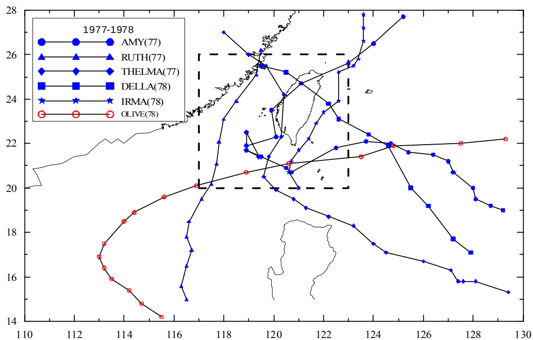
圖 3.5.2 (續 3) 歷年侵臺颱風路徑圖 (1977-1978 年)
