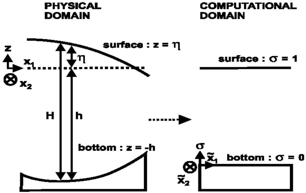
圖 4.1.1.2 垂直方向之 \sigma 座標系統 (from COHERENS User Documentation)
