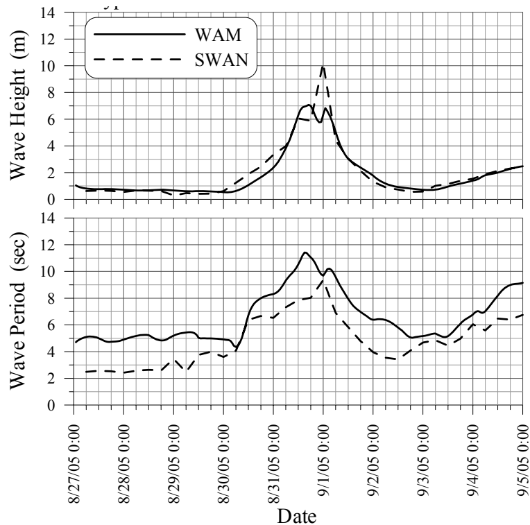
圖 3.1.20 泰利颱風侵襲時蘇澳港之推算波浪與觀測波浪比較圖
