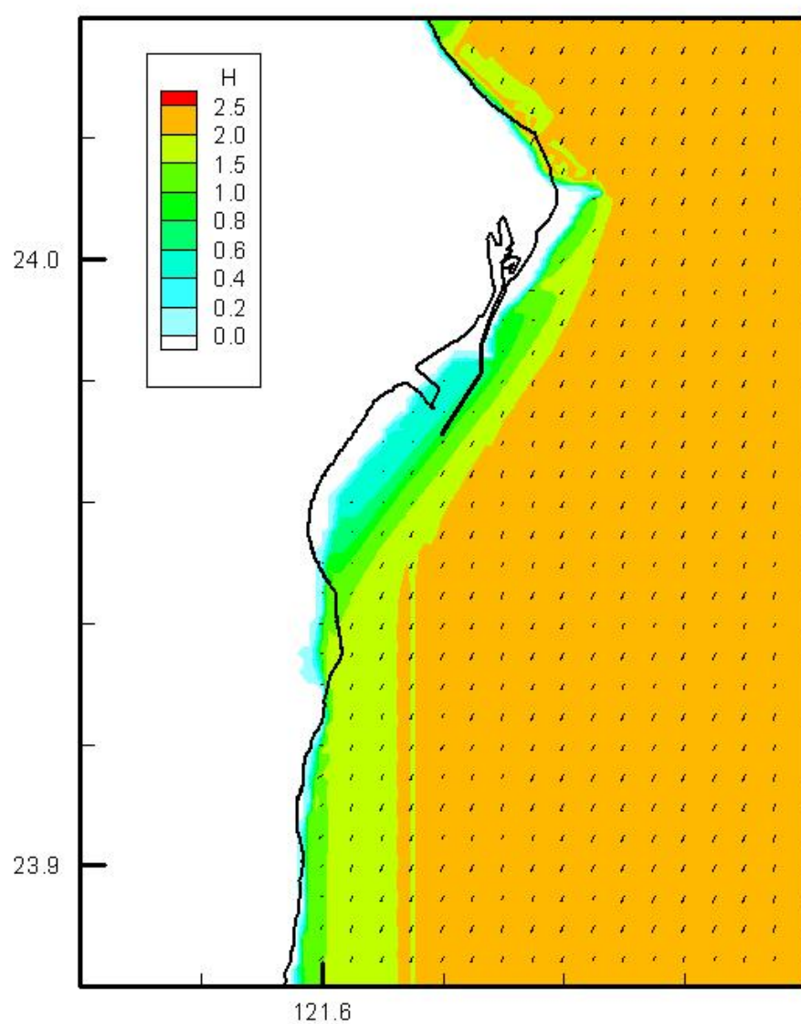
圖3.2.32 近岸區域波浪模式模擬區域F之波高及波向分佈
