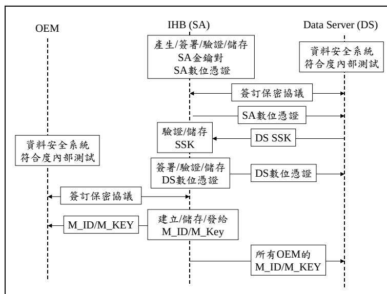
圖 9 SA 參與 S63 資料保護計畫的運作程序
