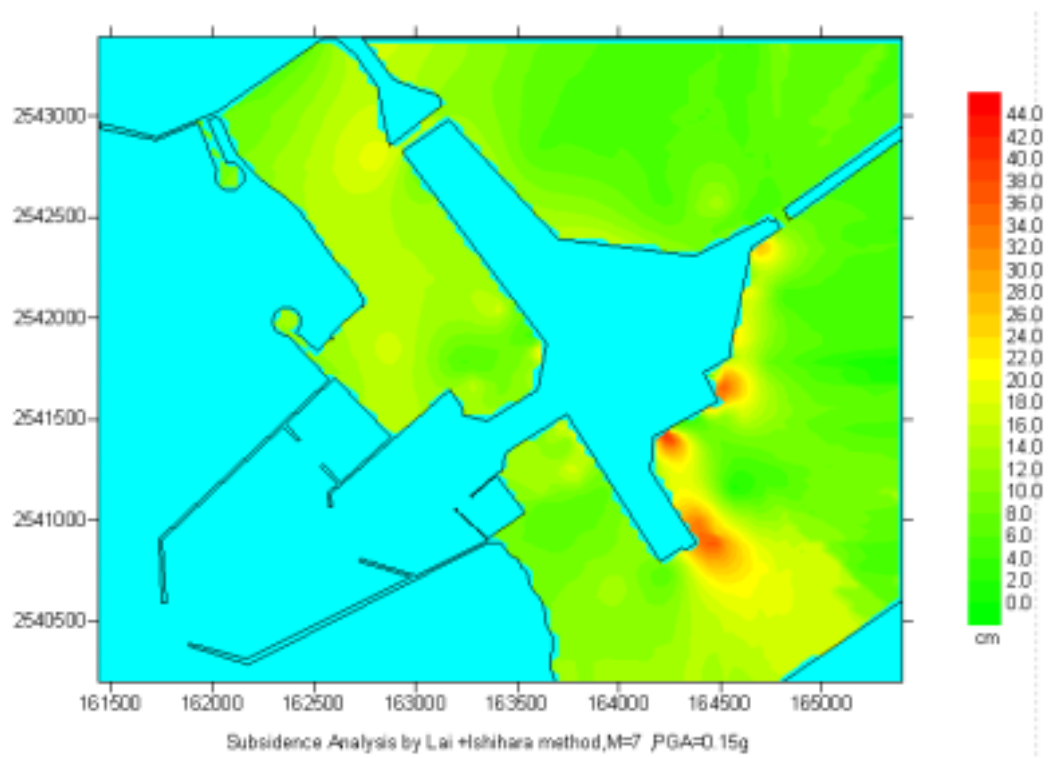
圖 6-30 安平港區地震下陷分析成果圖
