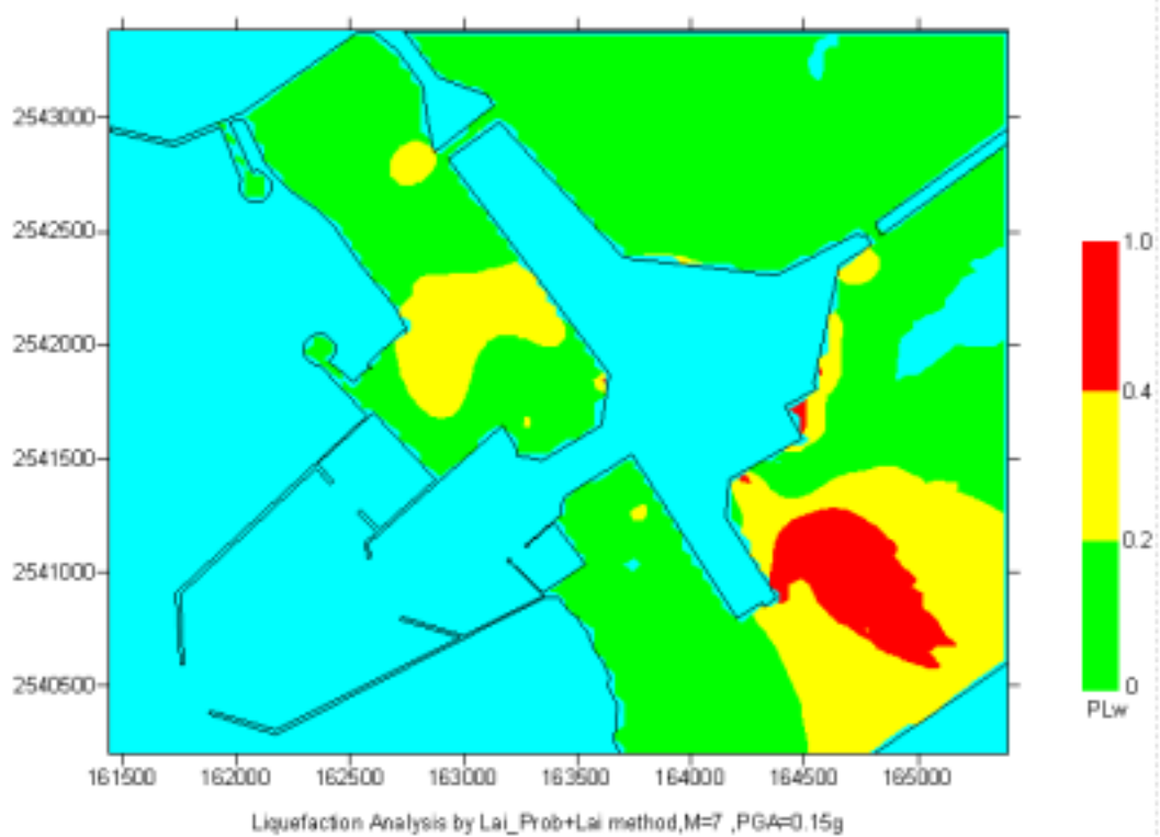
圖 6-27 安平港區 Lai_Prob+Lai 法全區液化危險性指數分佈圖
