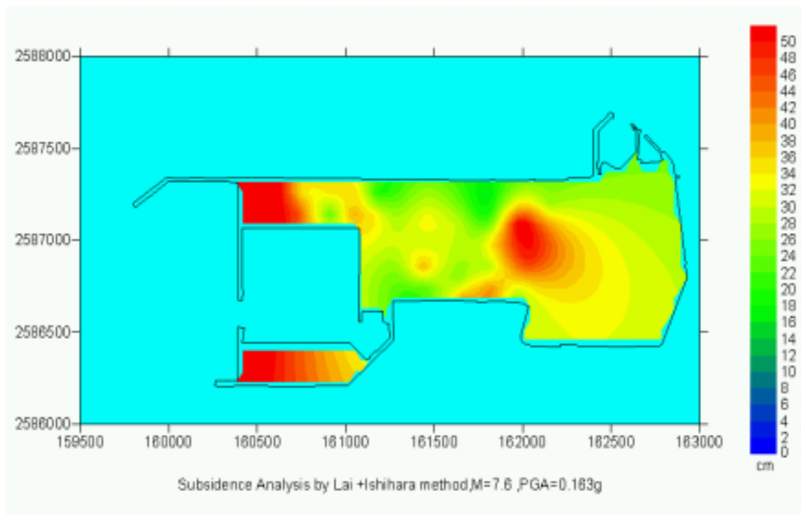
圖 6-15 布袋港區地震下陷分析成果圖
