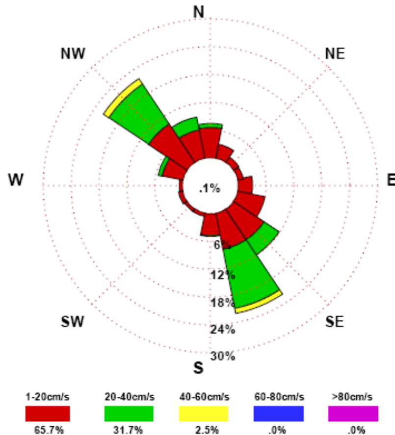
圖 8.4.88 2005 年 11 月安平港 1 站海流玫瑰圖
