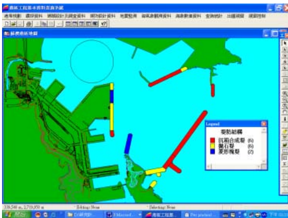
圖10-5 蘇澳港區堤防結構型式主題圖
