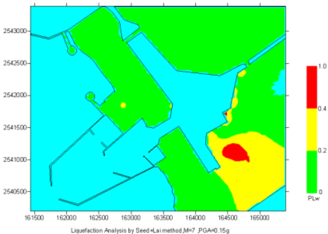
圖 6-24 安平港區 Seed+Iwasaki 法全區液化危險性指數分佈圖
