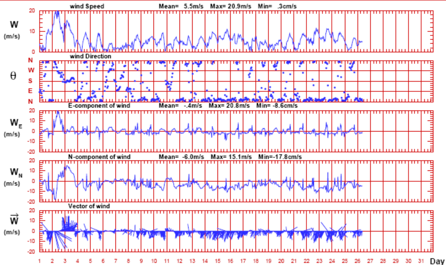
圖 4.4.73 2005 年 10 月安平港測站 1 風歷線圖
