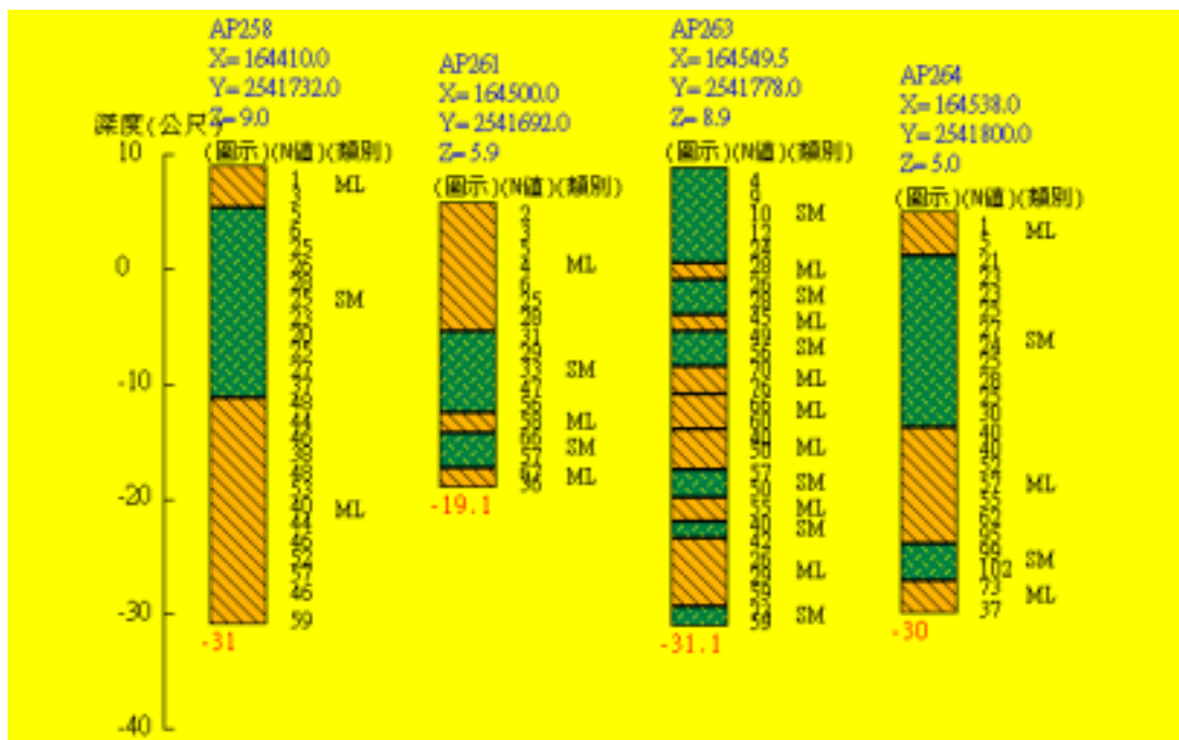
圖 6-19 安平港區鑽孔柱狀圖
