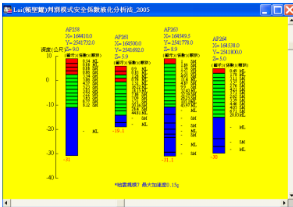
圖 6-28 安平港區 Lai 抗液化安全係數柱狀圖
