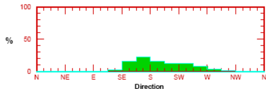
圖7.4.98 2005年11月安平港測站1波高波向及週期方塊圖
