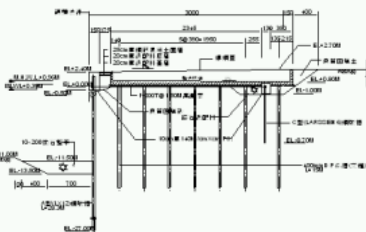
安平港奇美23號碼頭斷面圖
