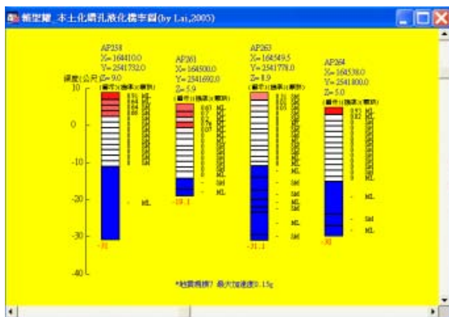
圖 6-26 安平港區鑽孔 Lai 液化機率分析結果柱狀圖
