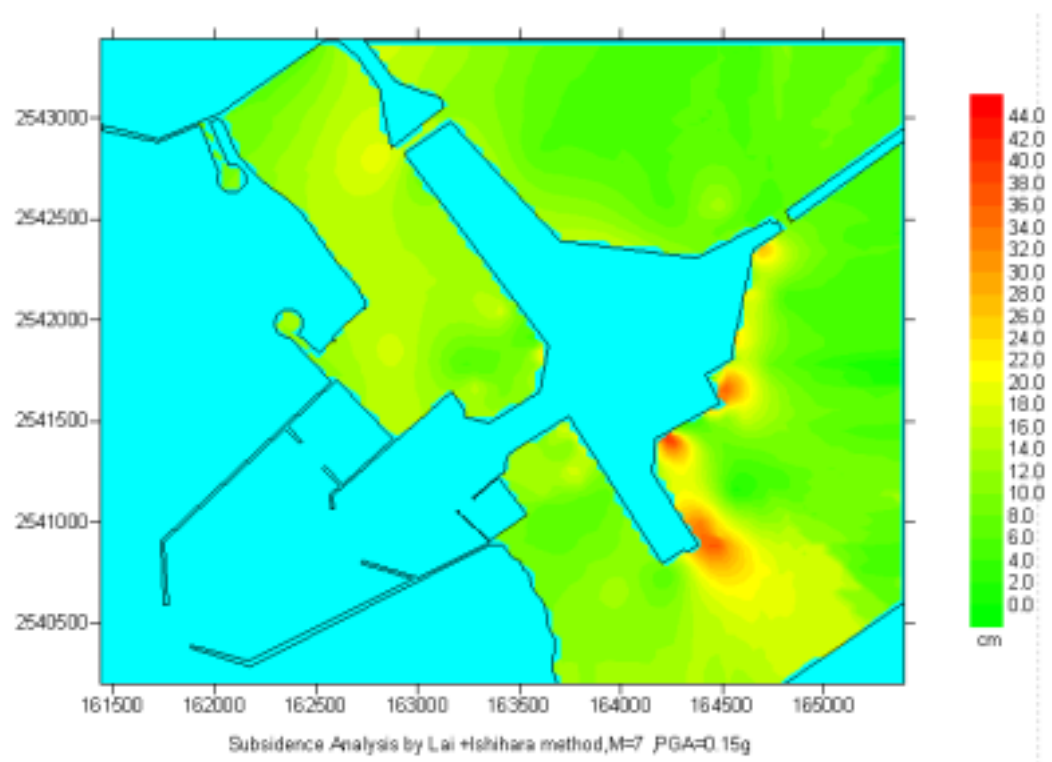
圖 6-30 地震下陷分析成果圖
