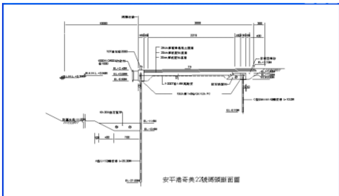
圖7-12 安平港區碼頭斷面圖之一
