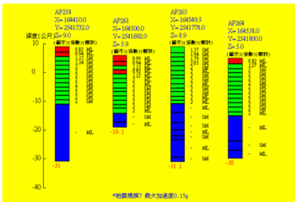
圖 6-23 安平港區 Seed 抗液化安全係數柱狀圖
