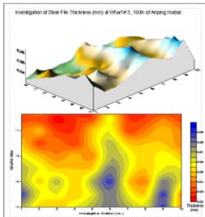
圖 8-16 安平港鋼板厚度調查成果展繪圖
