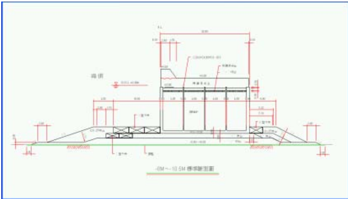
圖10-12 安平港區堤防斷面圖之一
