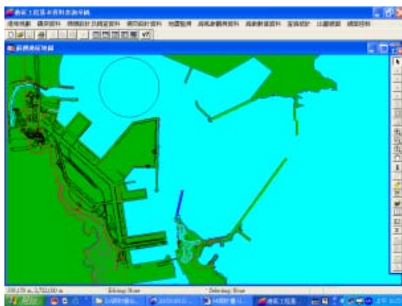
圖 3-2 蘇澳港區地圖圖層及所開發之選單列
