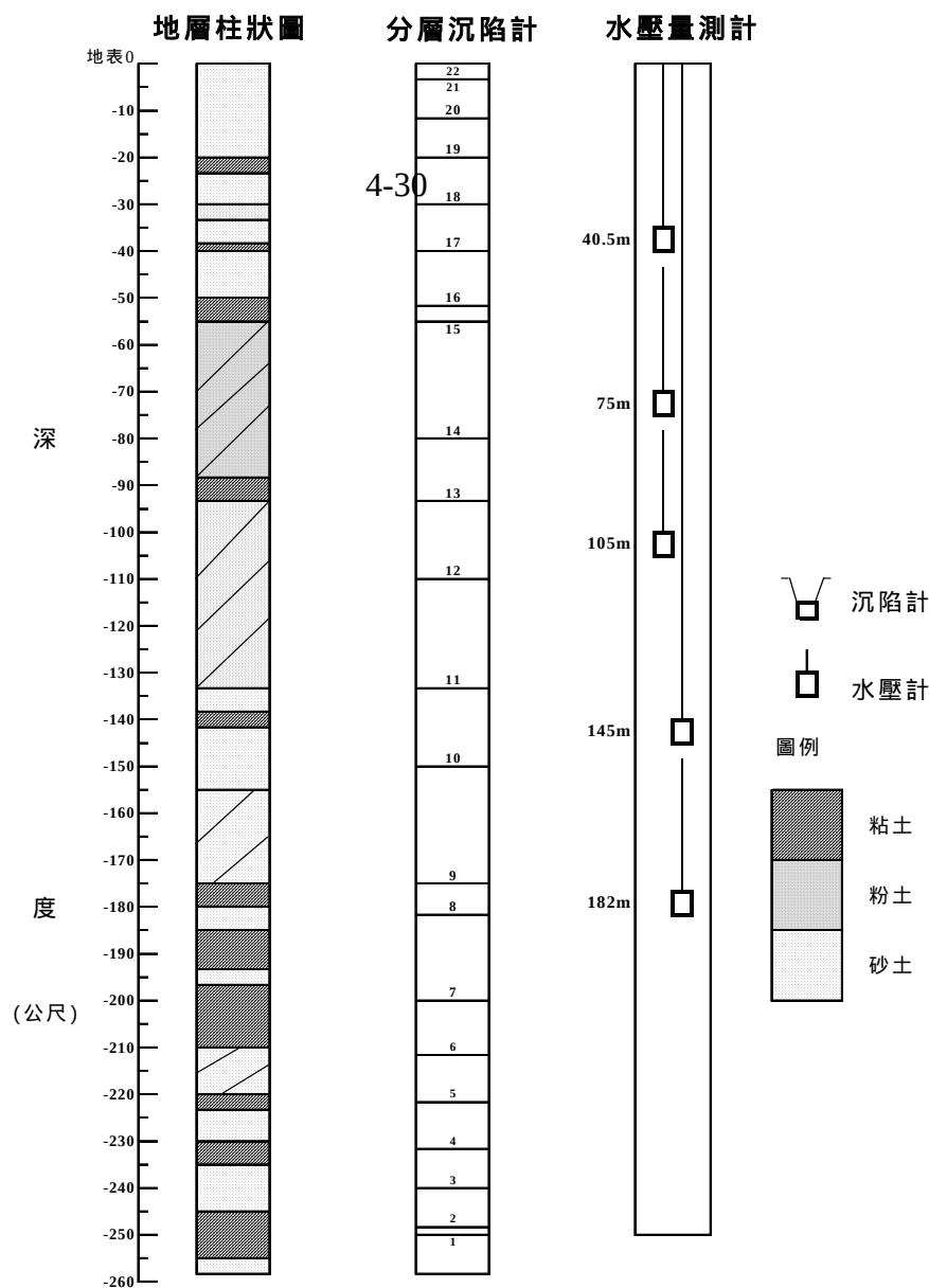
圖 4-15 安平港分層沉陷及水壓觀測站土層柱狀圖
