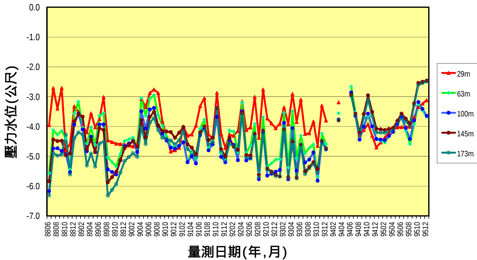
圖 4-20 臺中港分層水位變化圖(手動量測)
