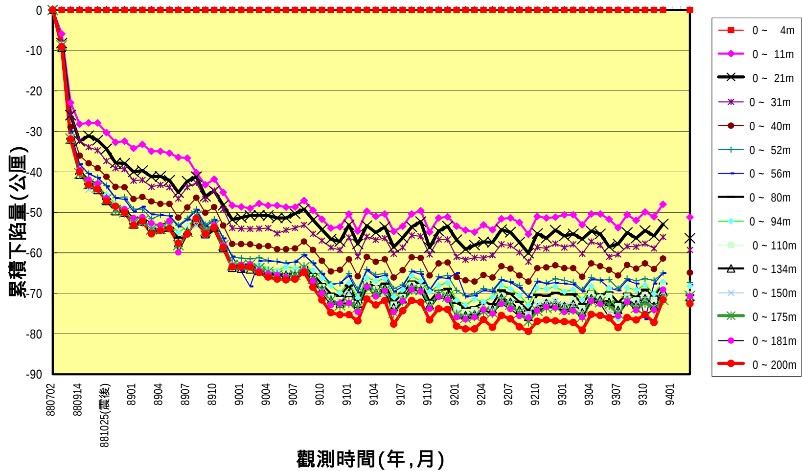
圖 4-17 安平港分層累積下陷量圖
