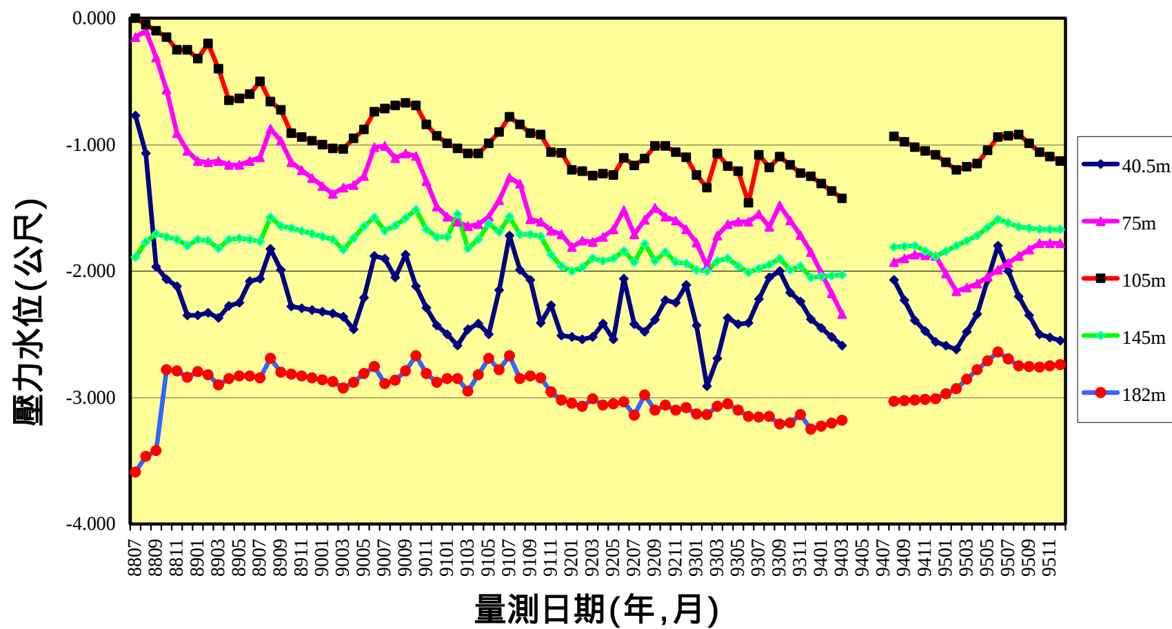
圖 4-16 安平港分層水位變化圖(手動量測)
