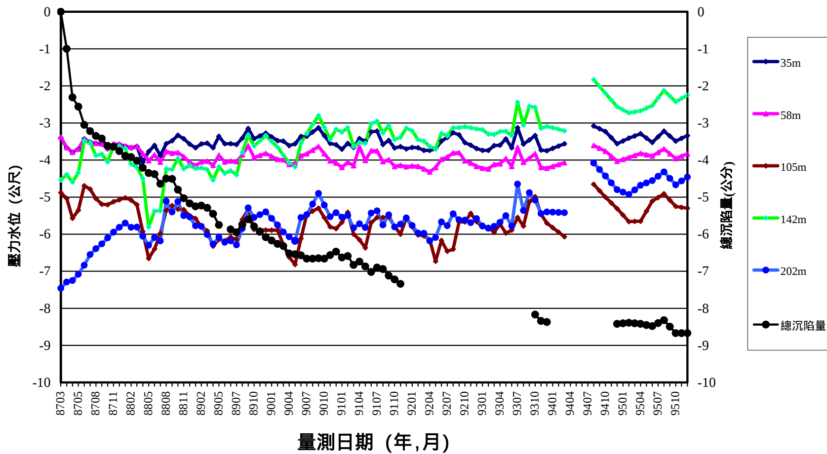
圖 4-14 大鵬灣地層下陷與地下水位變化觀測圖
