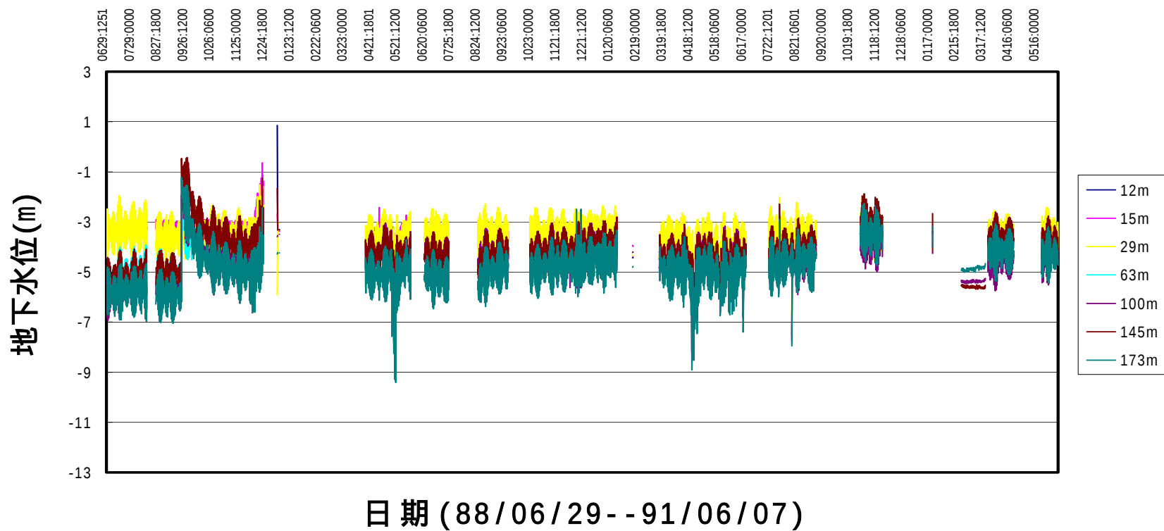
圖 4-19 臺中港分層水位變化圖(自記式)
