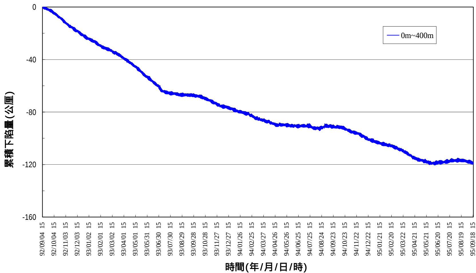
圖 4-8 布袋港 400 公尺永久水準點累積沉陷量(92/09~95/09)
