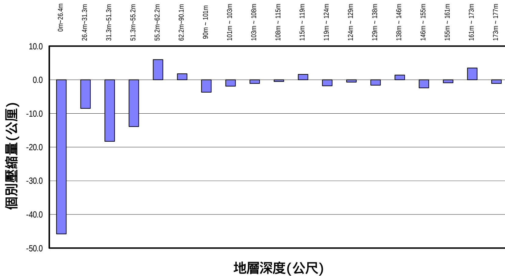
圖 4-12 大鵬灣分層個別下陷量圖
