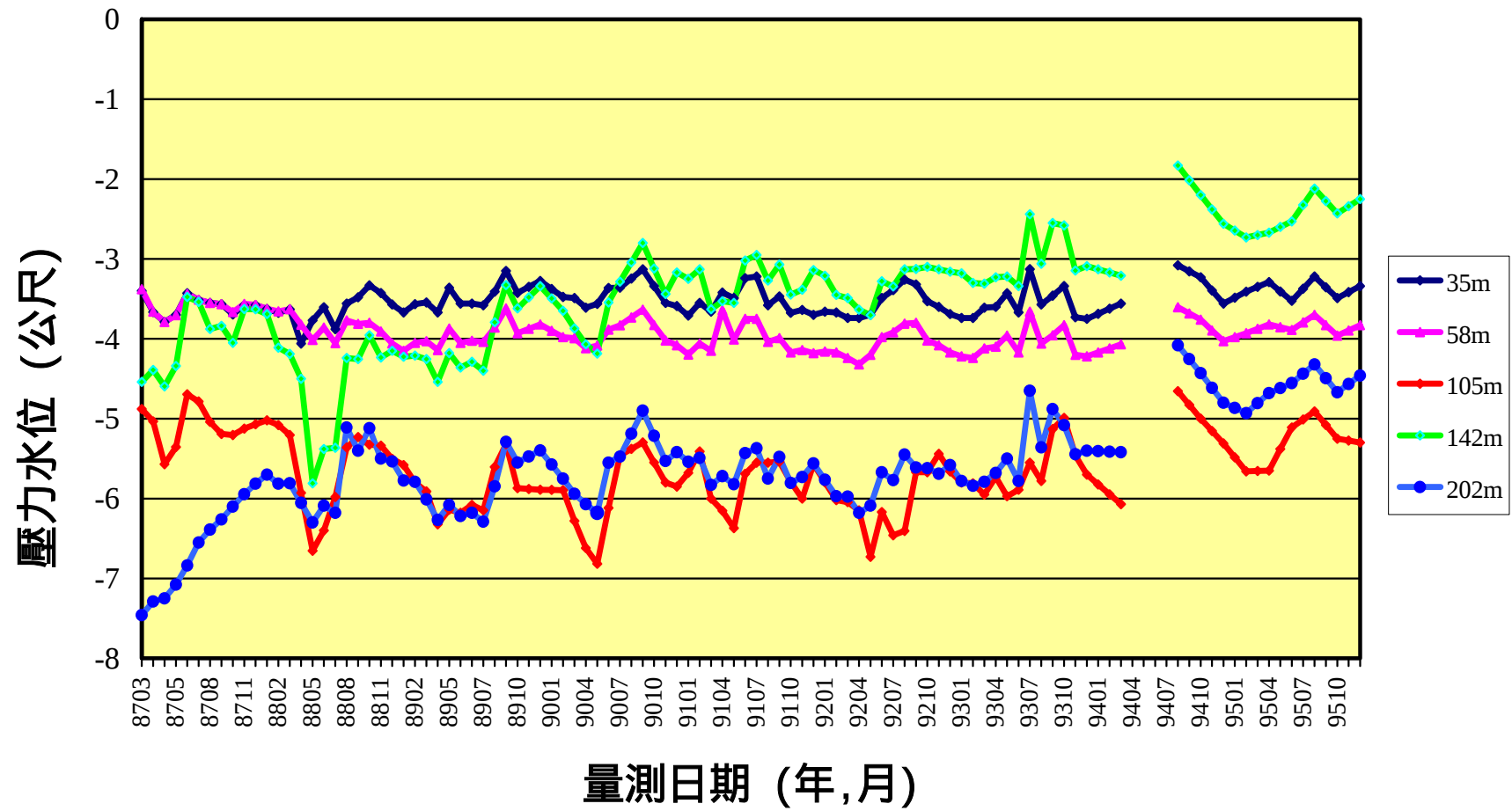
圖 4-11 大鵬灣分層水位變化圖(手動量測)
