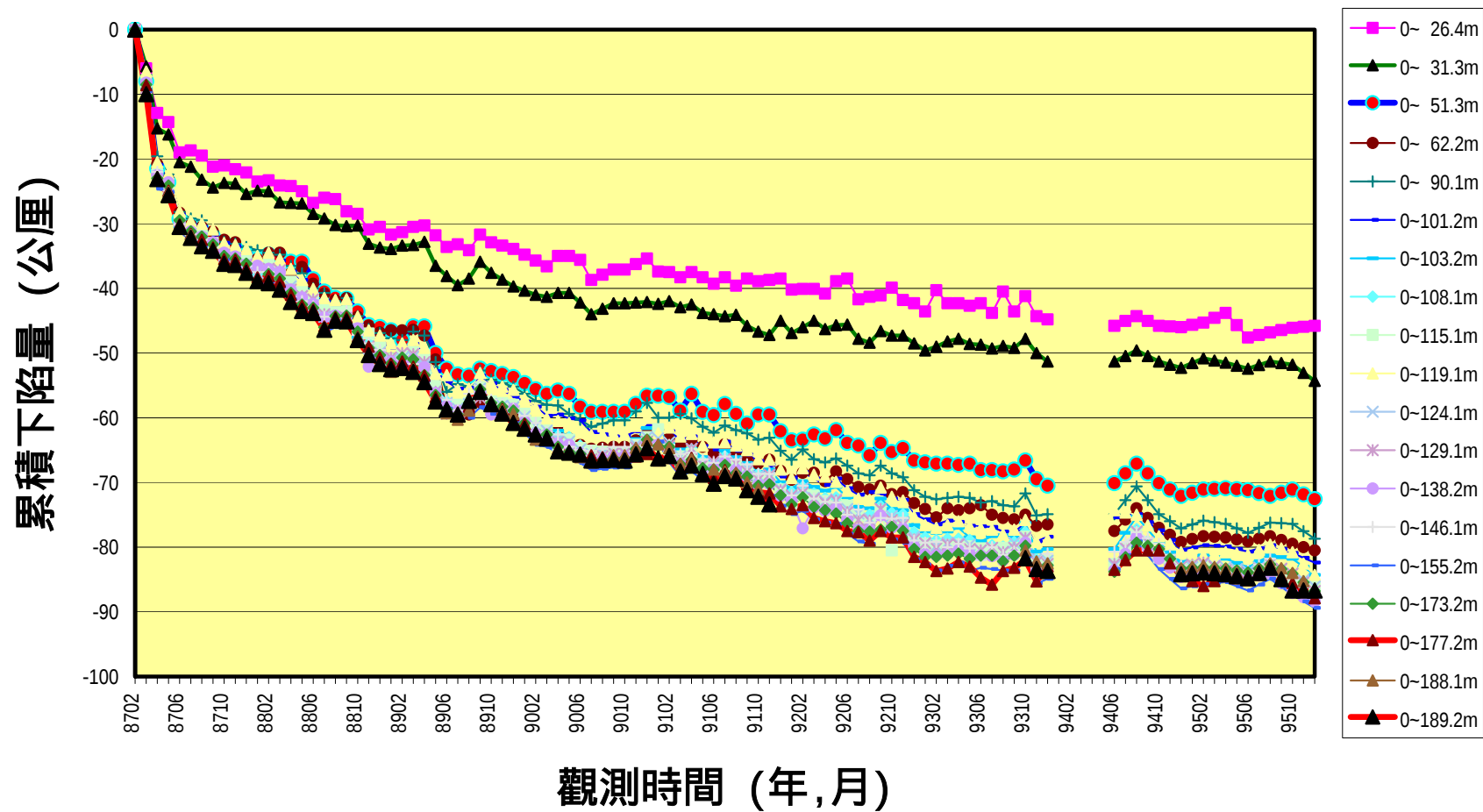
圖 4-13 大鵬灣地層分層下陷觀測圖
