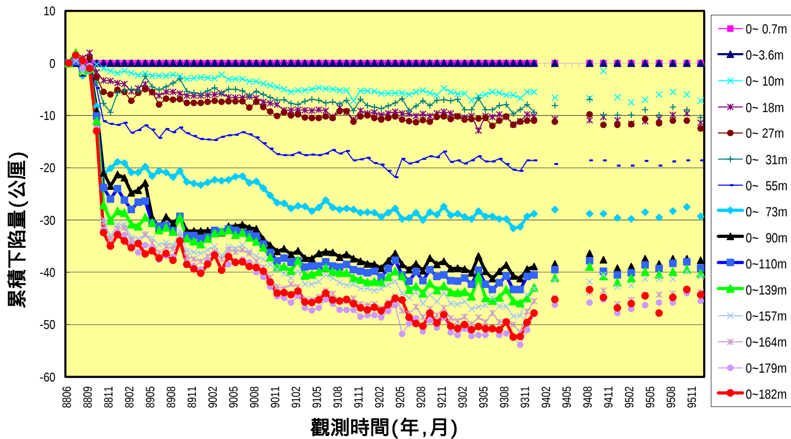
圖 4-21 臺中港分層累積下陷量圖(200m)
