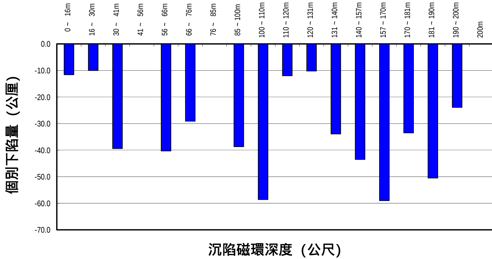
圖 4-6 布袋港分層個別下陷量圖
