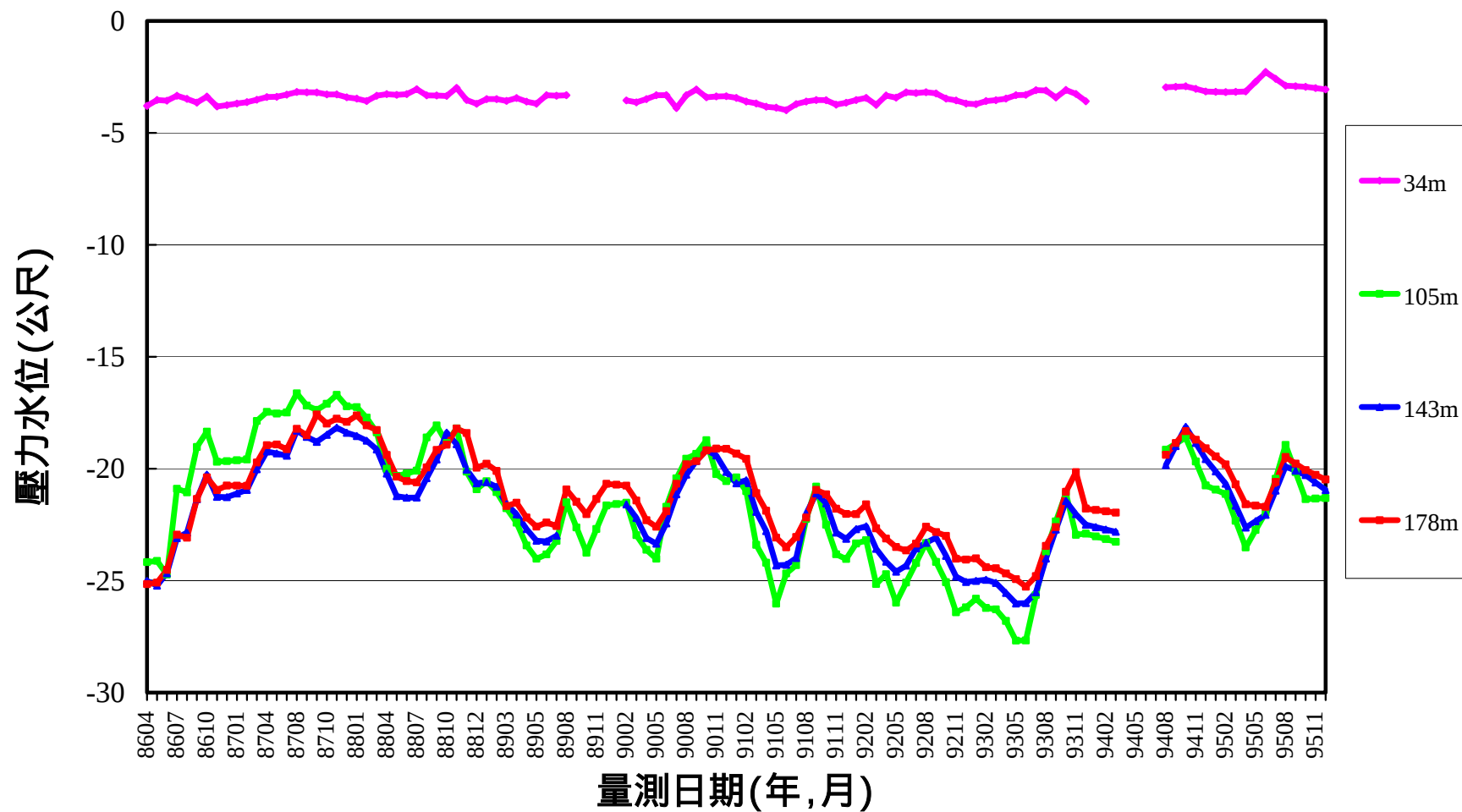
圖 4-4 布袋港分層水位變化圖(手動量測)
