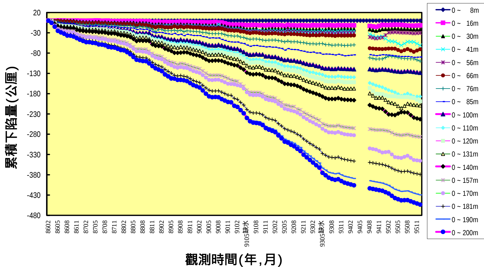
圖 4-7 布袋港分層累積下陷量圖(200m)
