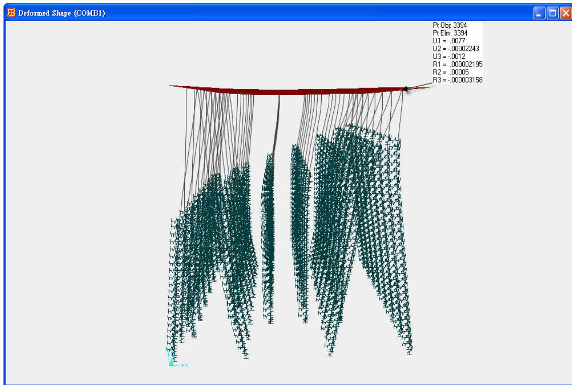
圖 6.6 水平震度 K_h=0.1 棧橋式碼頭變位示意圖
