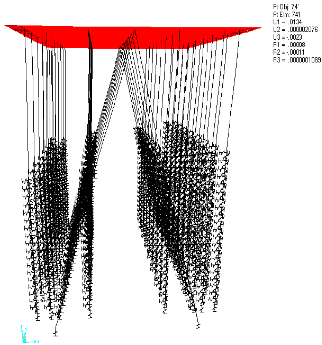
圖 5.11 水平震度 K_h=0.1 斜樁棧橋式碼頭變位示意圖
