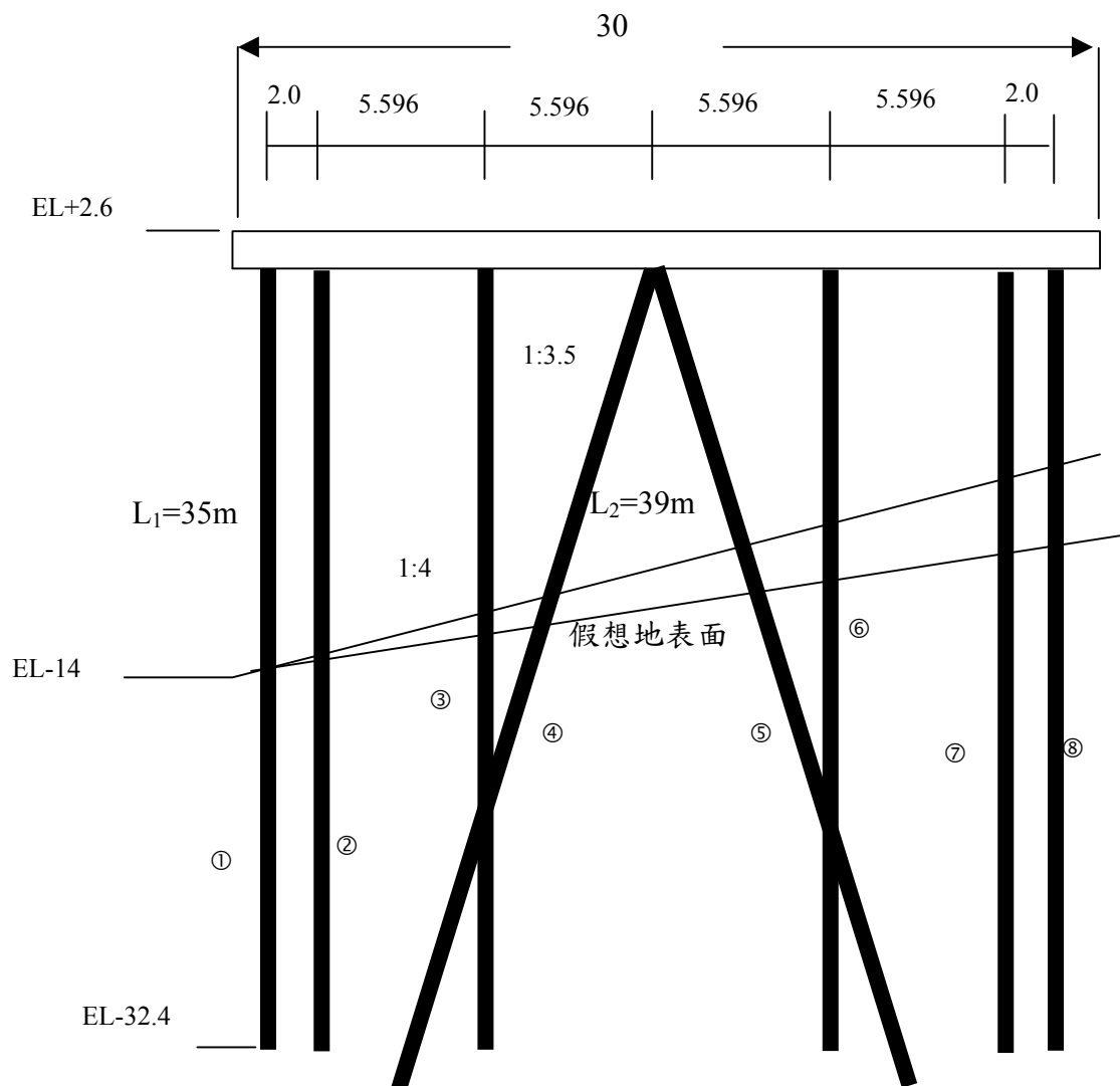
圖 4.4 斷面各樁長及編號示意圖
