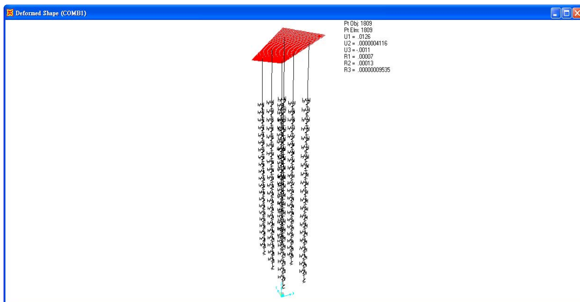
圖 5.7 水平震度 K_h=0.1 碼頭變位示意圖
