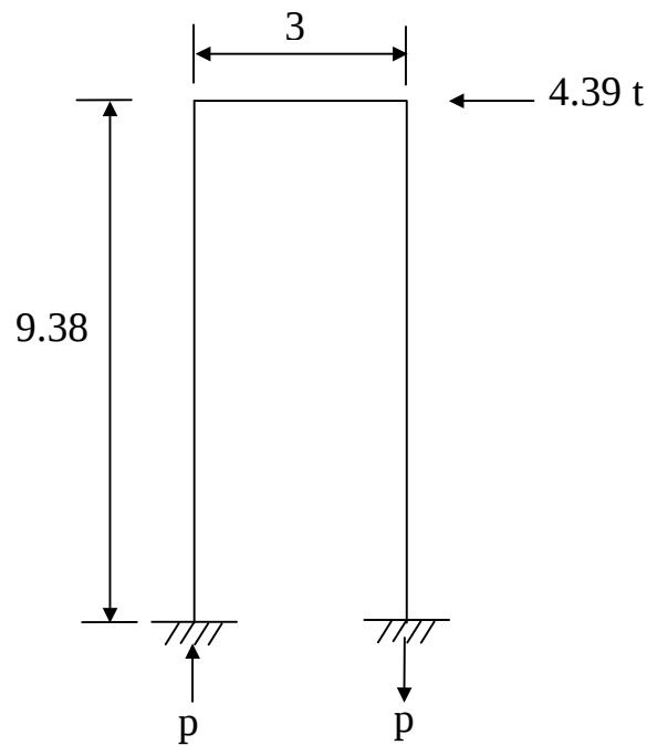
圖 5.5 地震力產生之樁頭彎矩及軸力示意圖
