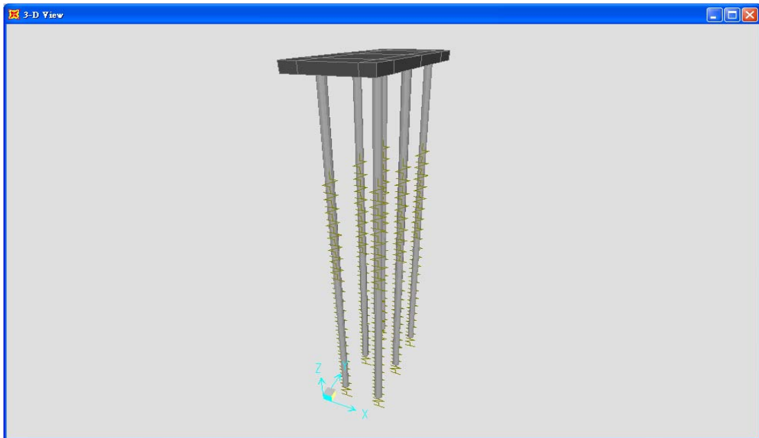
圖 5.6 直樁棧橋式碼頭 SAP2000 模型及土壤彈簧示意圖
