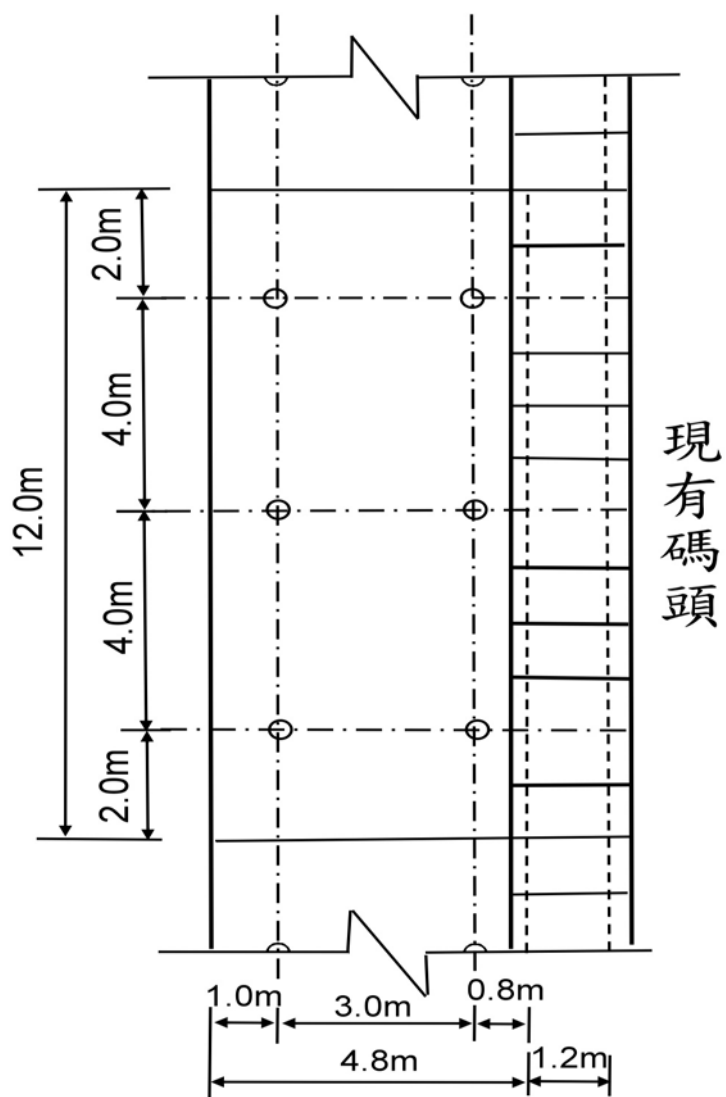
圖 5.2 上部結構及樁之配置示意圖
