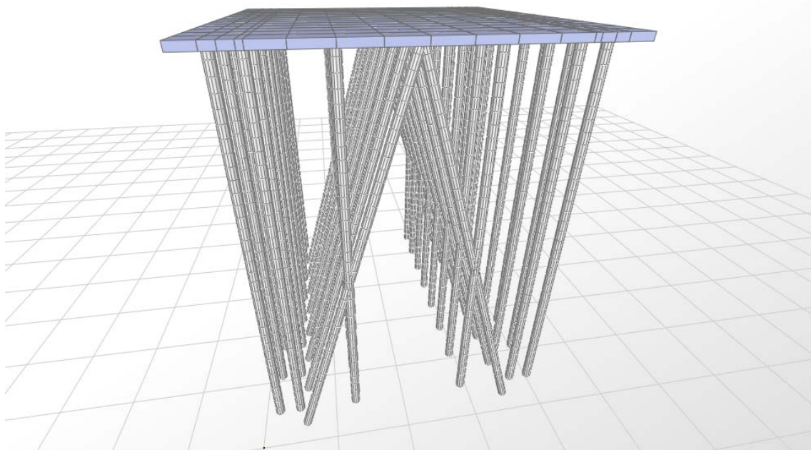
圖 5.9 斜樁棧橋式碼頭 SAP2000 模型示意圖
