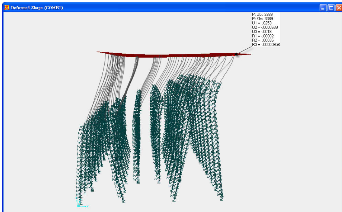
圖 6.7 水平震度 K_h=0.32 棧橋式碼頭變位示意圖
