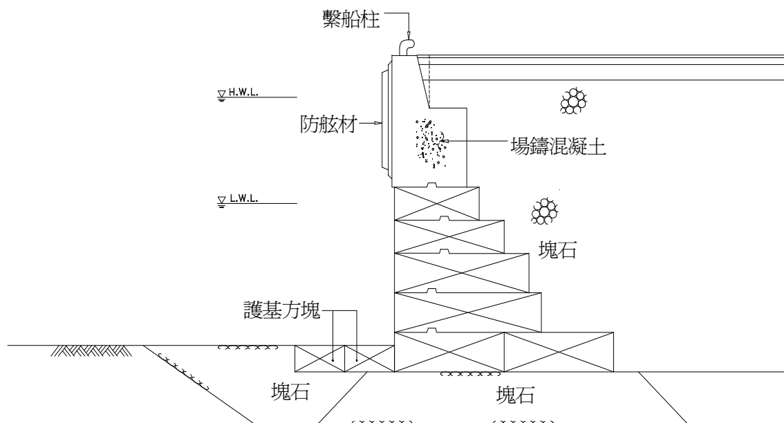
圖 2.3 方塊式碼頭
