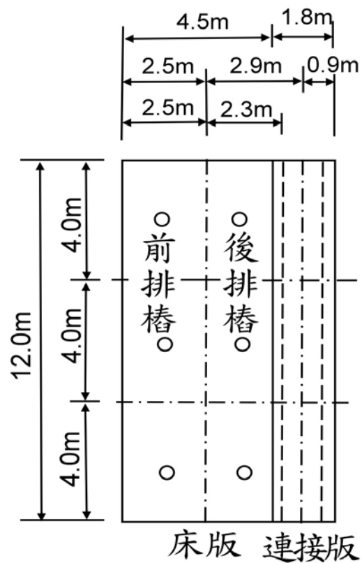
圖 5.4 各樁荷重分配區域示意圖
