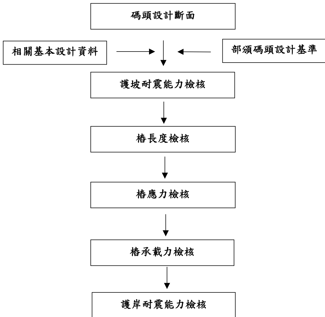
圖 4.1 棧橋式碼頭耐震能力評估項目與流程圖
