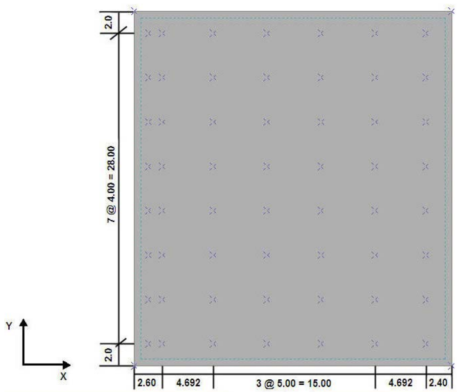
圖 6.3 碼頭面分析單元相關尺寸示意圖
