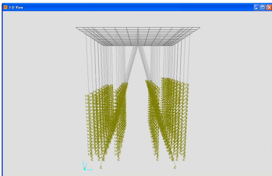
圖 5.10 斜樁棧橋式碼頭 SAP2000 土壤彈簧模擬示意圖
