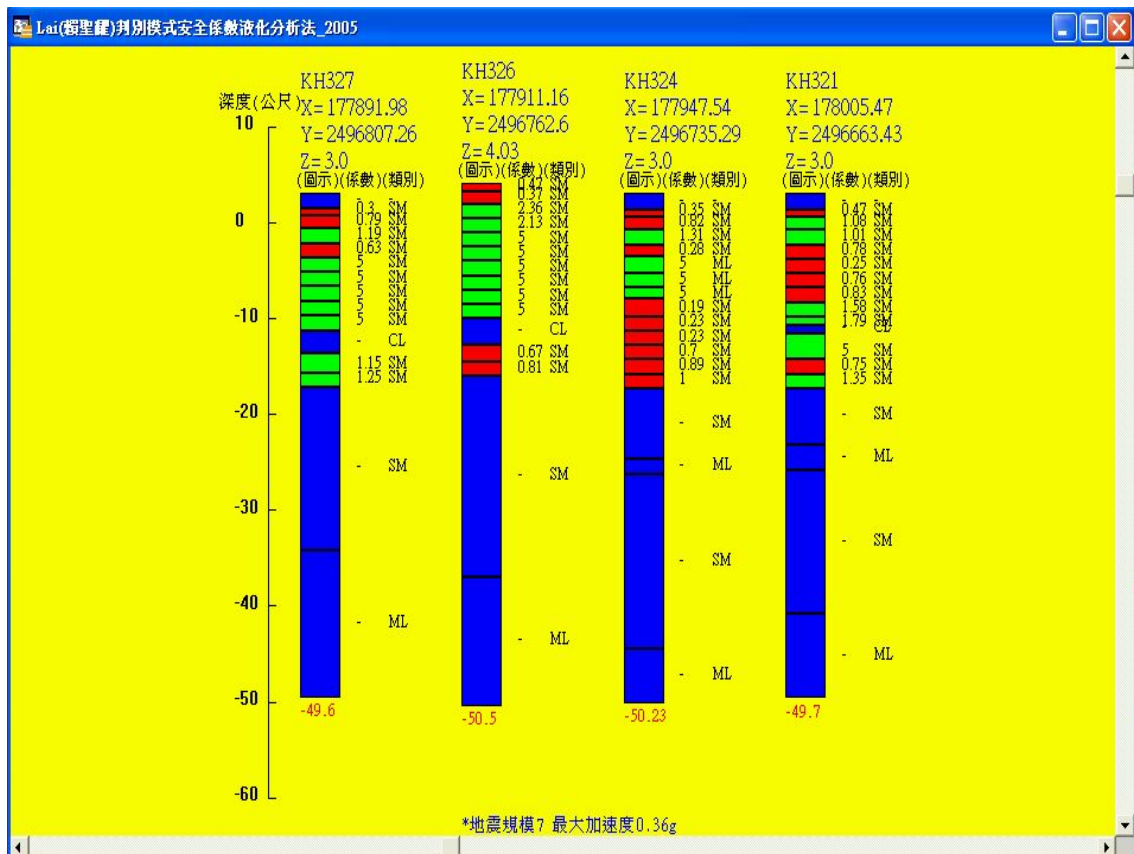
圖 6.9 水平震度 K_h=0.36 土層液化深度柱狀圖
