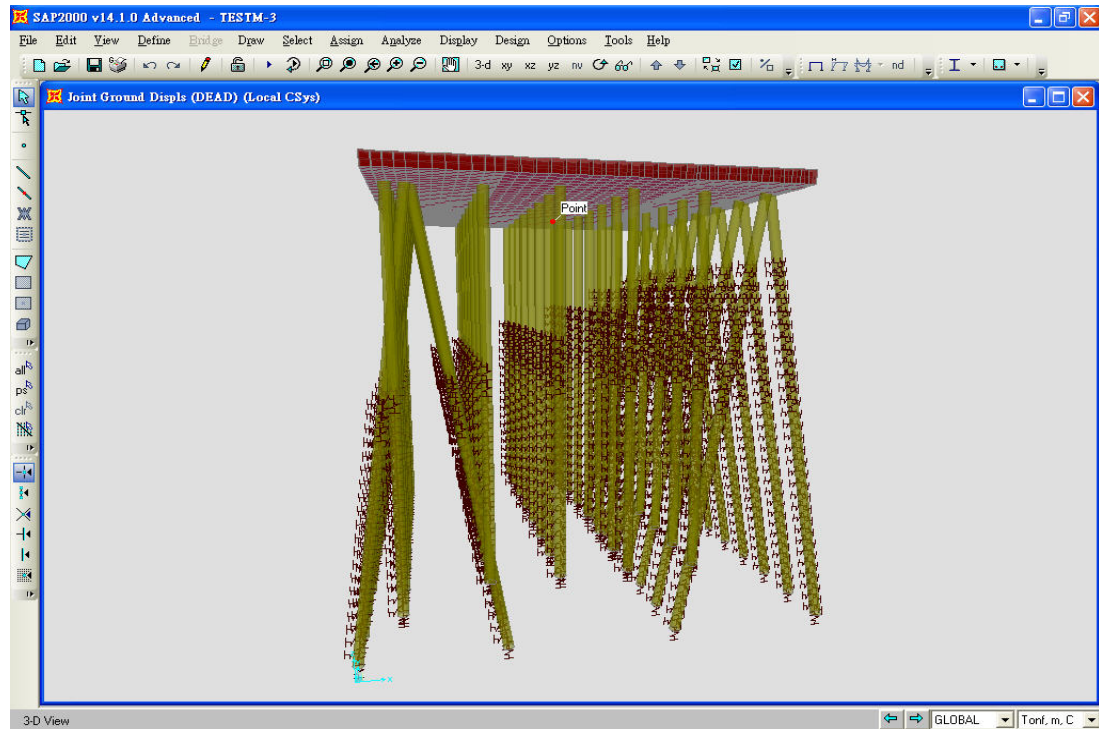
圖 6.5 棧橋式碼頭 SAP2000 土壤彈簧模擬示意圖
