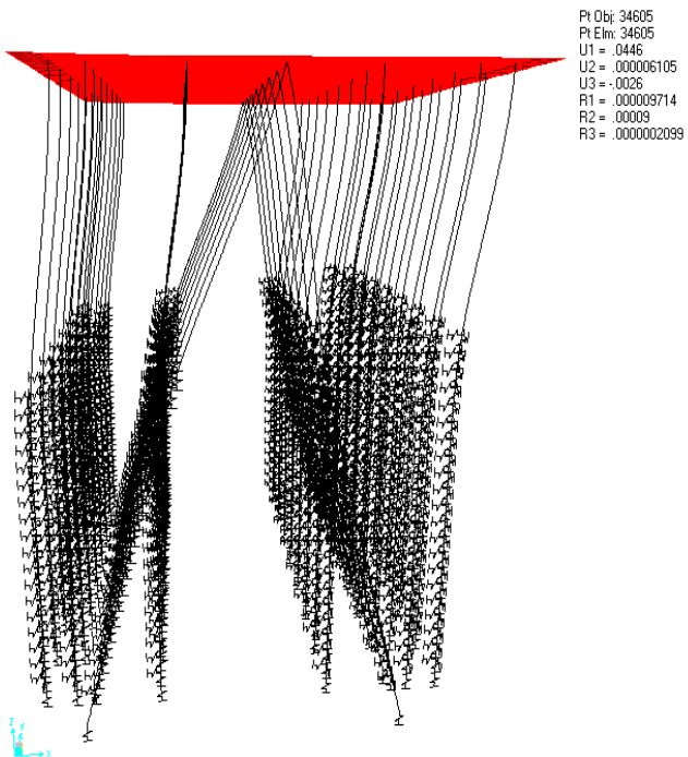
圖 5.12 水平震度 K_h=0.33 斜樁棧橋式碼頭變位示意圖
