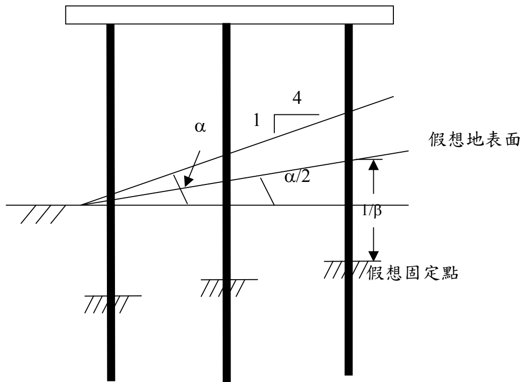
圖 4.3 假想地表面示意圖
