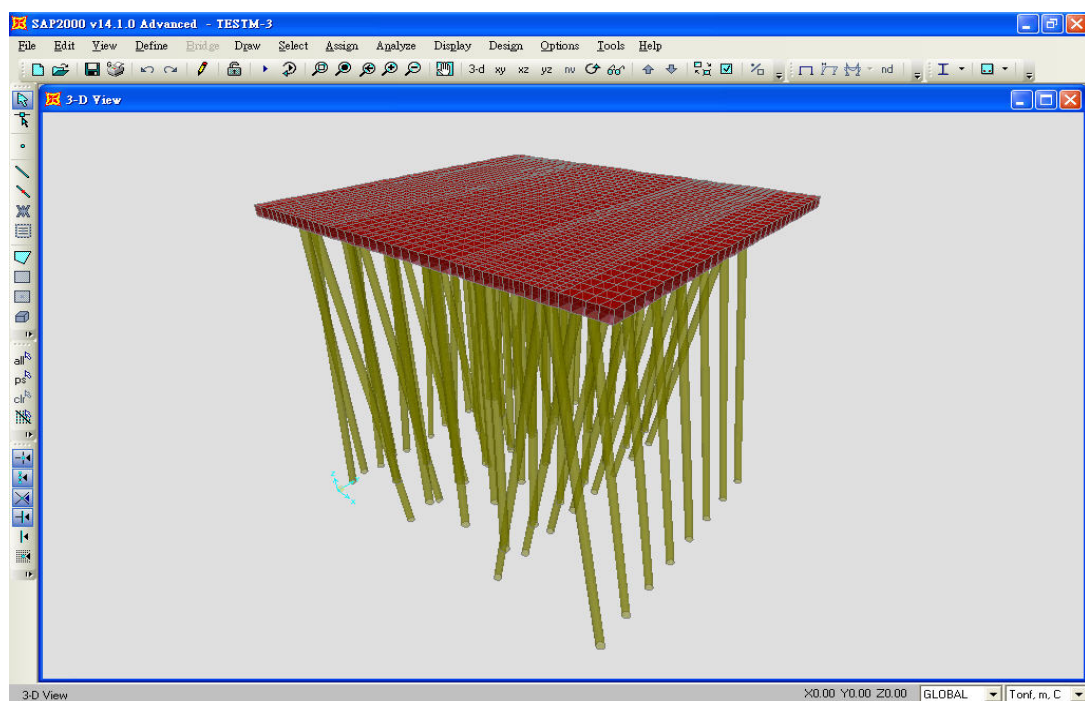
圖 6.4 棧橋式碼頭 SAP2000 模型示意圖
