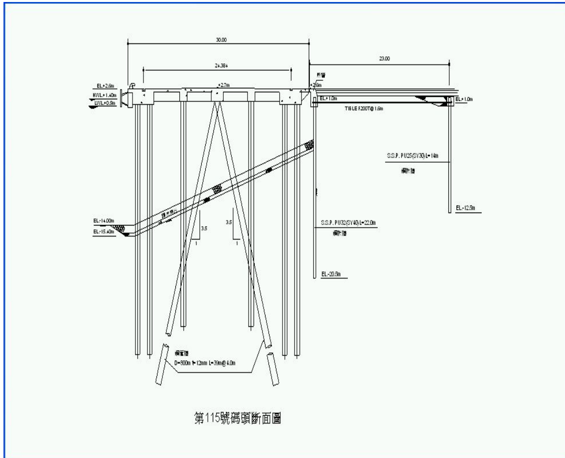
圖 4.2 碼頭斷面圖
