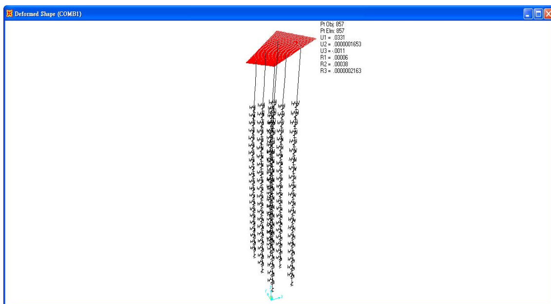
圖 5.8 水平震度 K_h=0.26 碼頭變位示意圖
