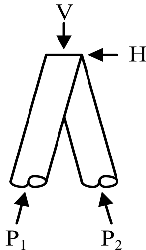
圖 4.6 群斜樁之軸力示意圖
