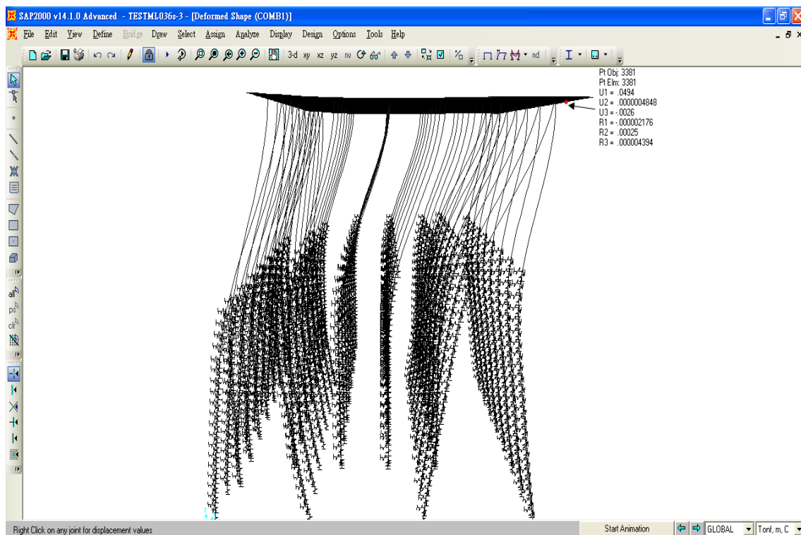
圖 6.10 水平震度 K_h=0.36 棧橋式碼頭變位示意圖
