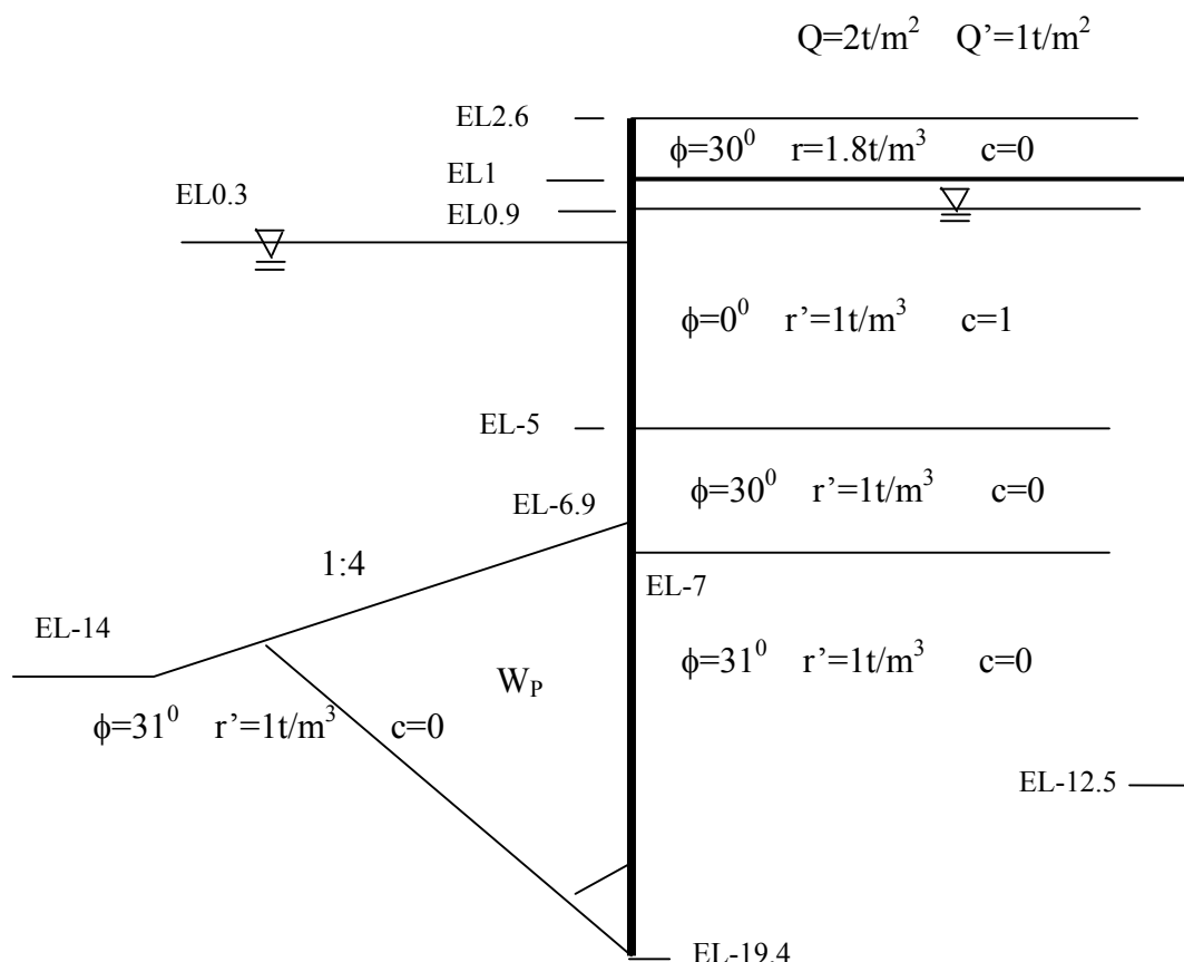
圖 4.7 護岸斷面及相關設計資料
