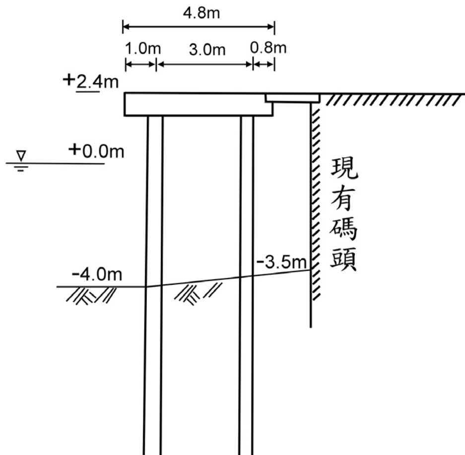
圖 5.1 直樁棧橋式碼頭斷面圖
