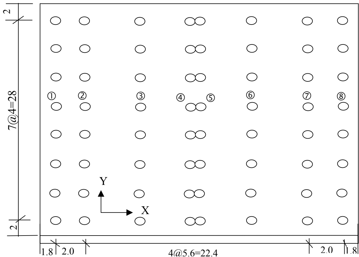
圖 4.5 棧橋式碼頭分析單元示意圖
