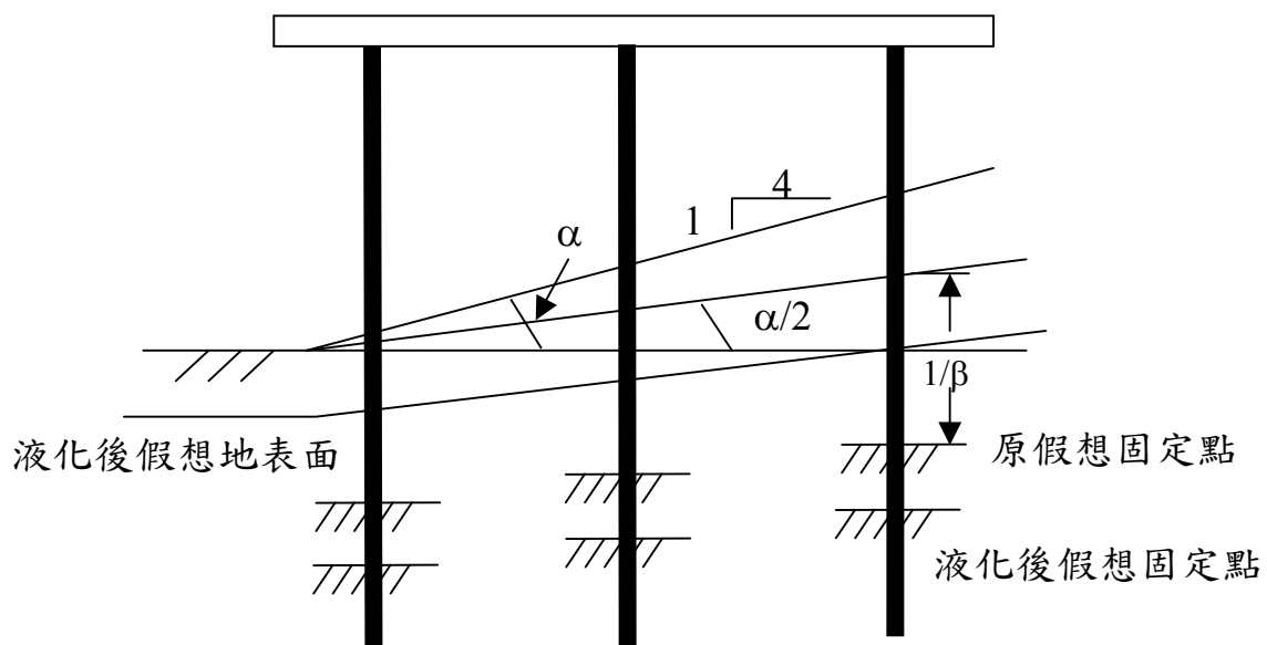
圖 4.8 液化後假想地表面示意圖
