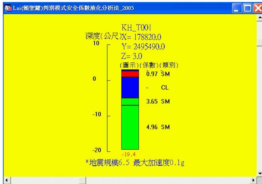
圖 4.7 土層液化深度柱狀圖
