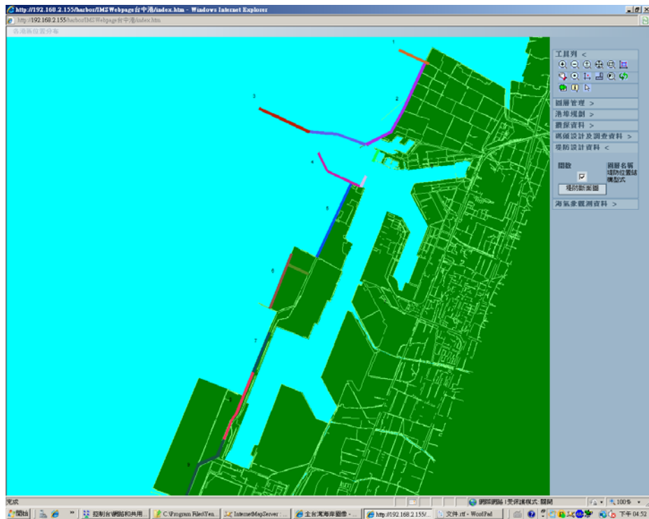
圖 2-18 堤防位置結構型式圖
