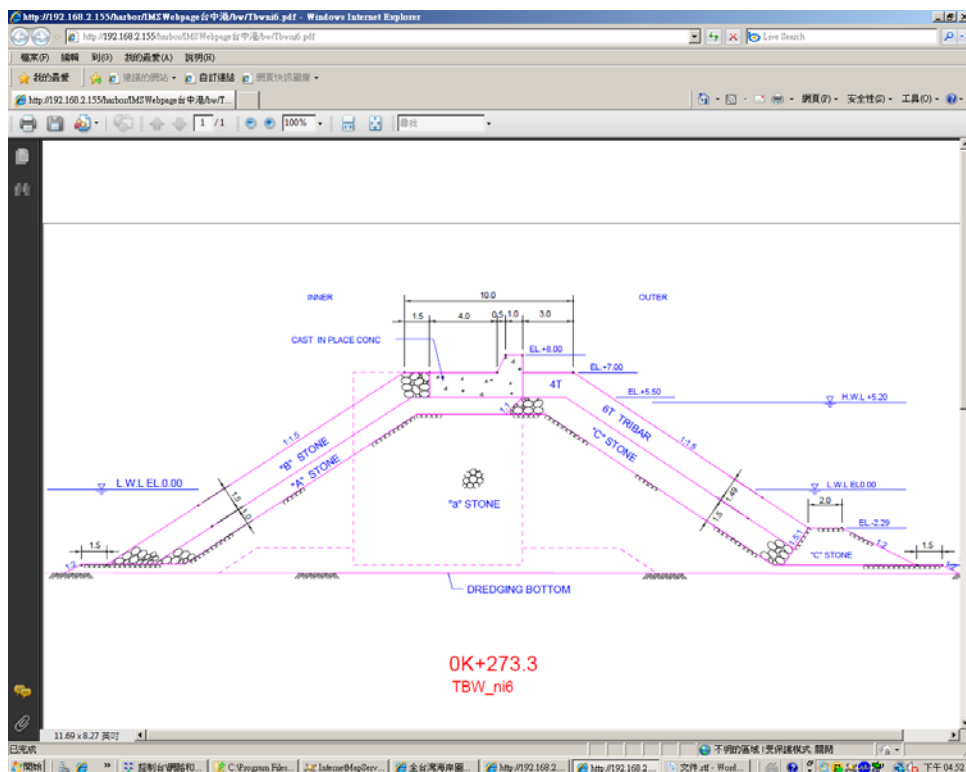
圖 2-19 堤防斷面圖
