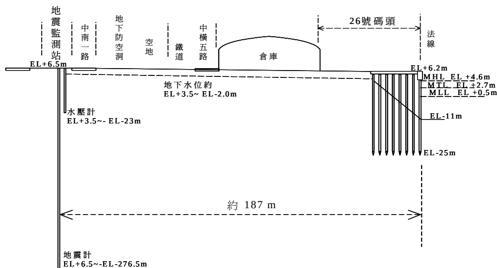
圖 5.3 測站相關測量結果斷面示意圖-臺中港範例
