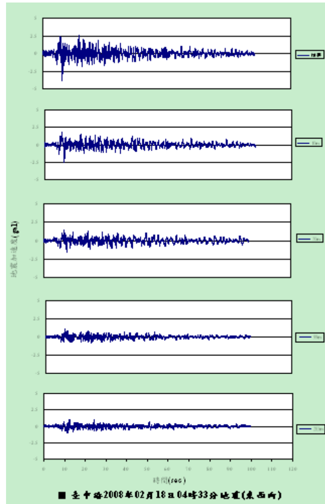
圖 5.16 臺中港地震引置之水壓反應記錄圖之一
