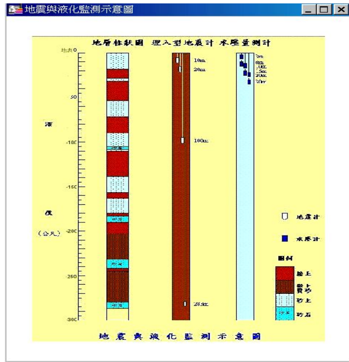
圖 5.9 臺中港區之地震監測系統設置示意圖
