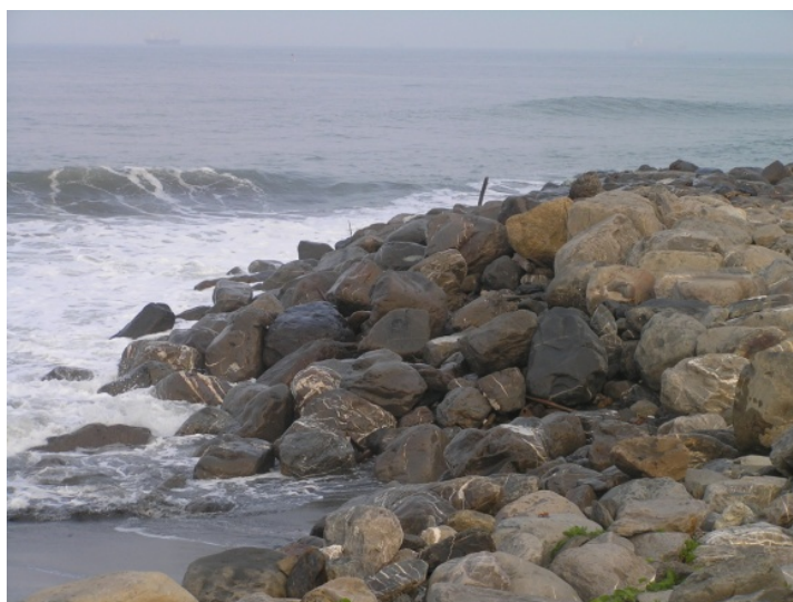
圖 5.52 旗津 拋石護岸
