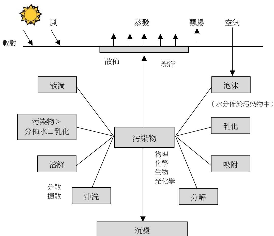
圖 2.4 污染物在海洋中之循環(資料來源：水體水質保護,楊萬發,1994 年)
