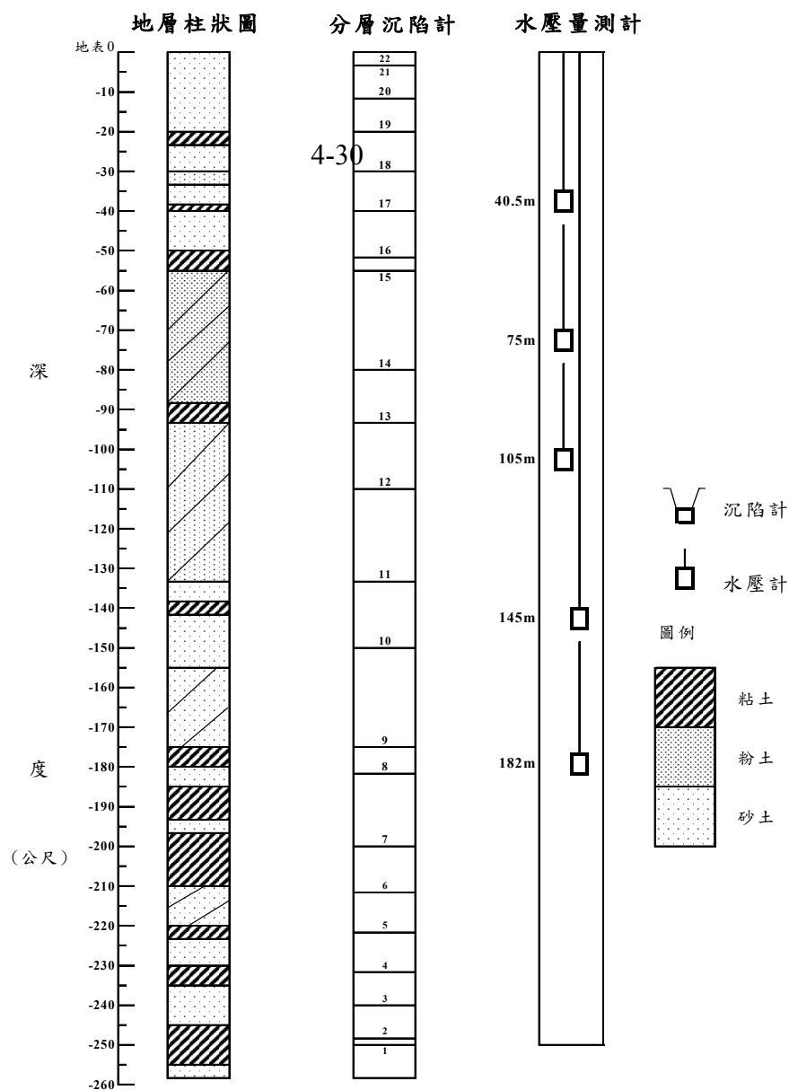
圖 4.15 安平港分層沉陷及水壓觀測站土層柱狀圖
