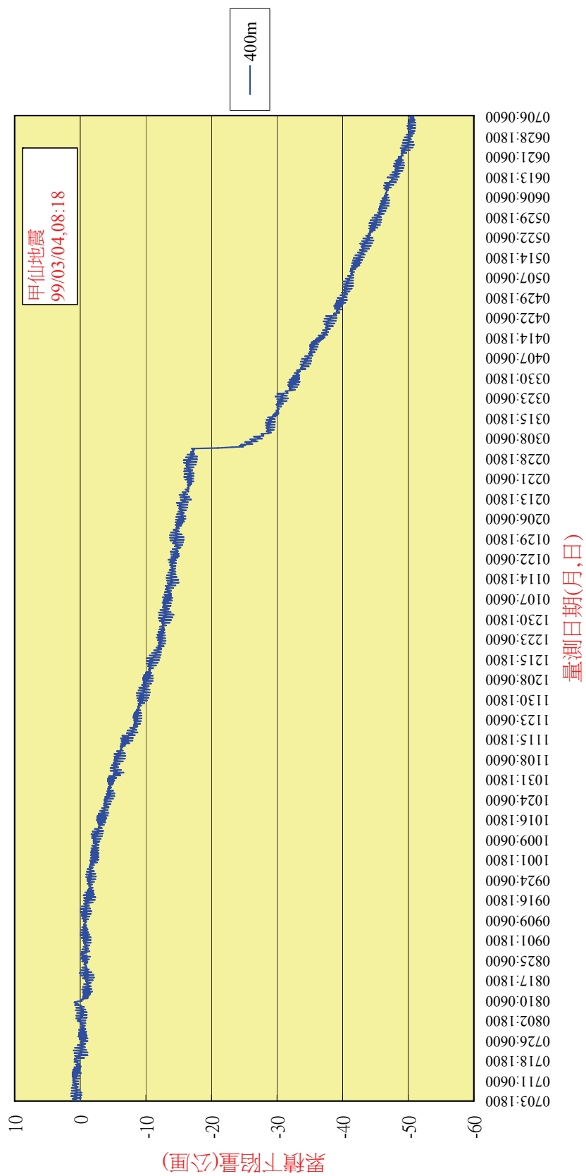
圖 4.8b 布袋港(400m)水準基準站累積下陷量圖(98/07/03~99/07/06)
