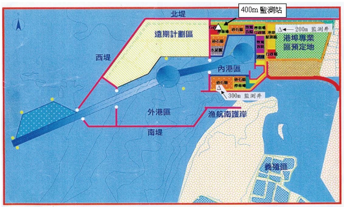
圖 3.6 布袋港監測站位置圖
