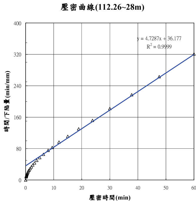
圖 4.9 矩形雙曲線壓密曲線圖
