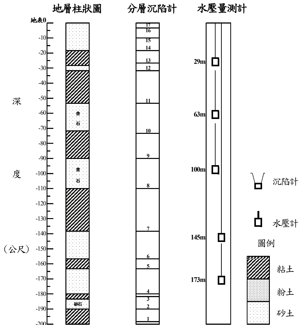
圖 4.18 臺中港分層沉陷及水壓觀測站土層柱狀圖
