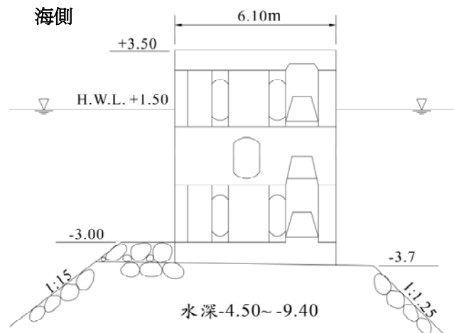
圖 4.2 混凝土塊堤設計斷面圖
