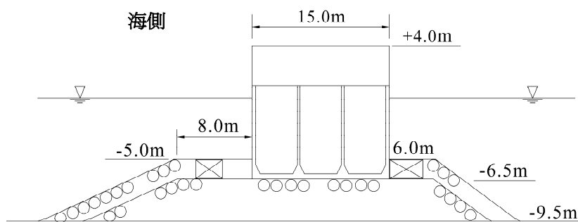
圖 4.3 合成堤設計斷面圖(邱永芳，2001)
