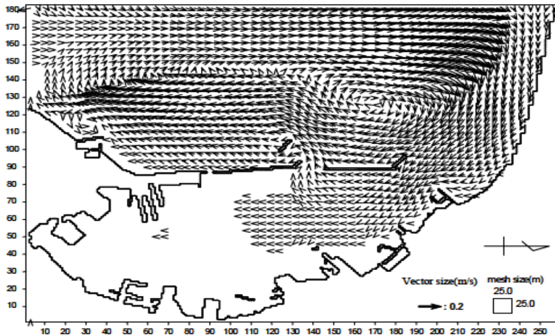
圖 2.2 殘差流流向圖
