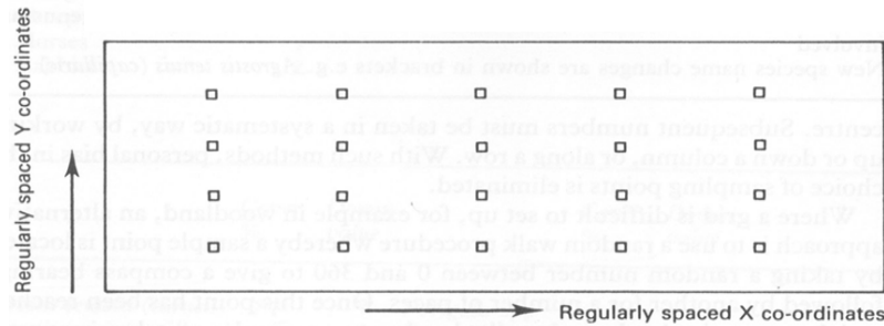
圖 3.2 系統取樣法
