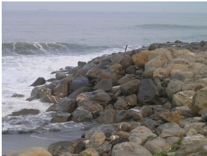
圖 4.23 旗津拋石護岸
