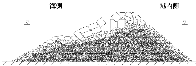
圖 4.1 拋石防波堤斷面圖(Quinn, 1961)
