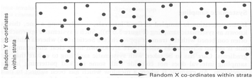
圖 3.3 分層取樣法
