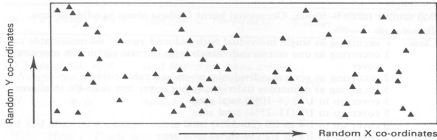
圖 3.1 隨機取樣法
