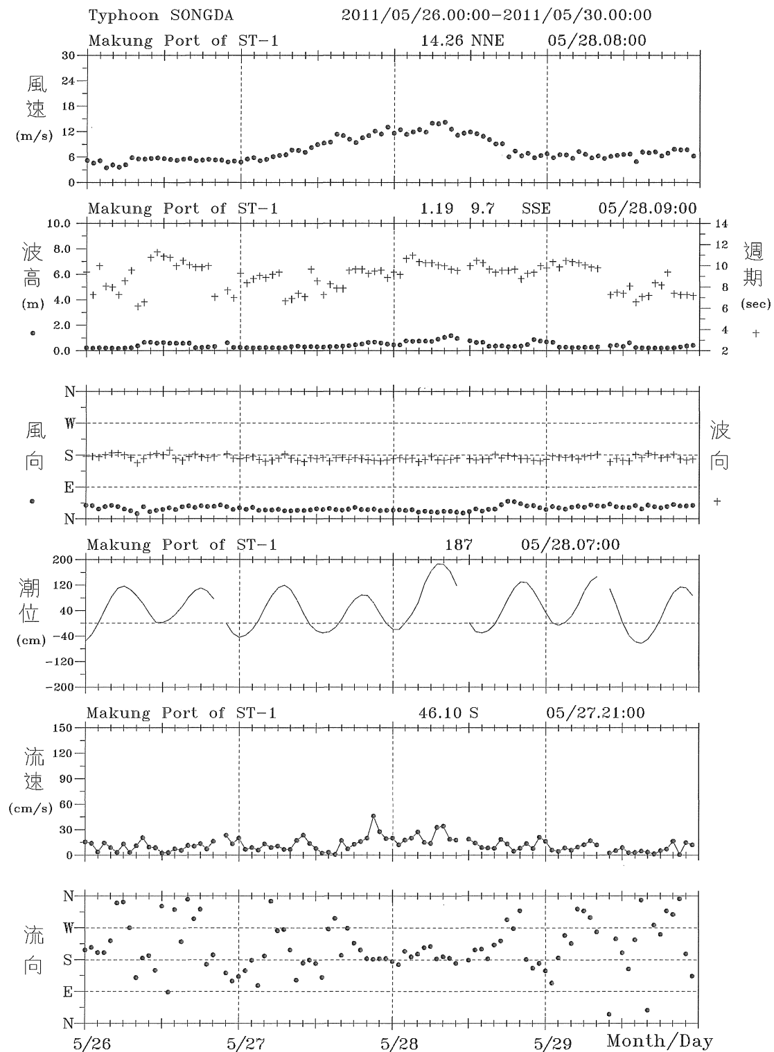
圖 6.3.12 2011 年 5 月桑達颱風馬公港測站風、潮、浪、流歷線圖
