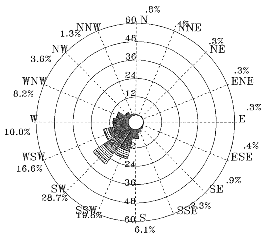
圖 4.2.31 歷年 9 月安平港 1 站波浪玫瑰圖
