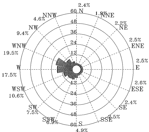
圖 4.2.22 歷年冬季安平港 1 站波浪玫瑰圖
