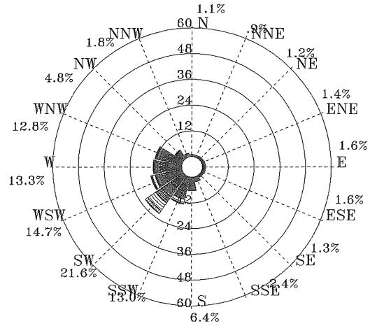
圖 4.2.36 歷年全年安平港 1 站波浪玫瑰圖
