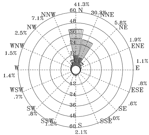
圖 4.2.4 歷年冬季臺北港1站波浪玫瑰圖
