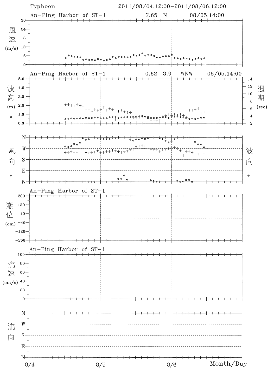
圖6.3.9 2011年8月梅花颱風安平港風、潮、浪、流歷線圖
