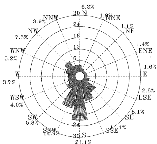
圖 5.2.39 2011 年冬季馬公港 1 站海流玫瑰圖
