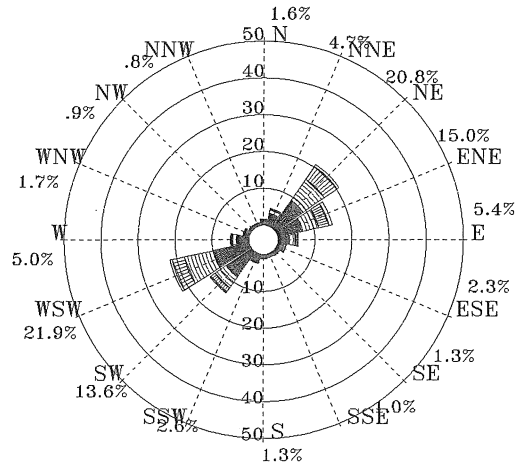
圖 5.2.13 歷年 9 月臺北港 1 站海流玫瑰圖
