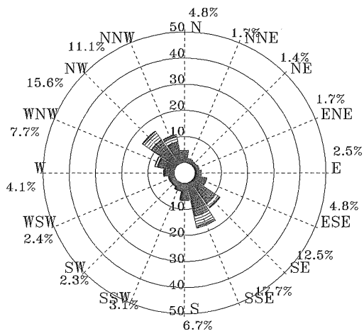
圖 5.2.30 歷年夏季安平港 1 站海流玫瑰圖
