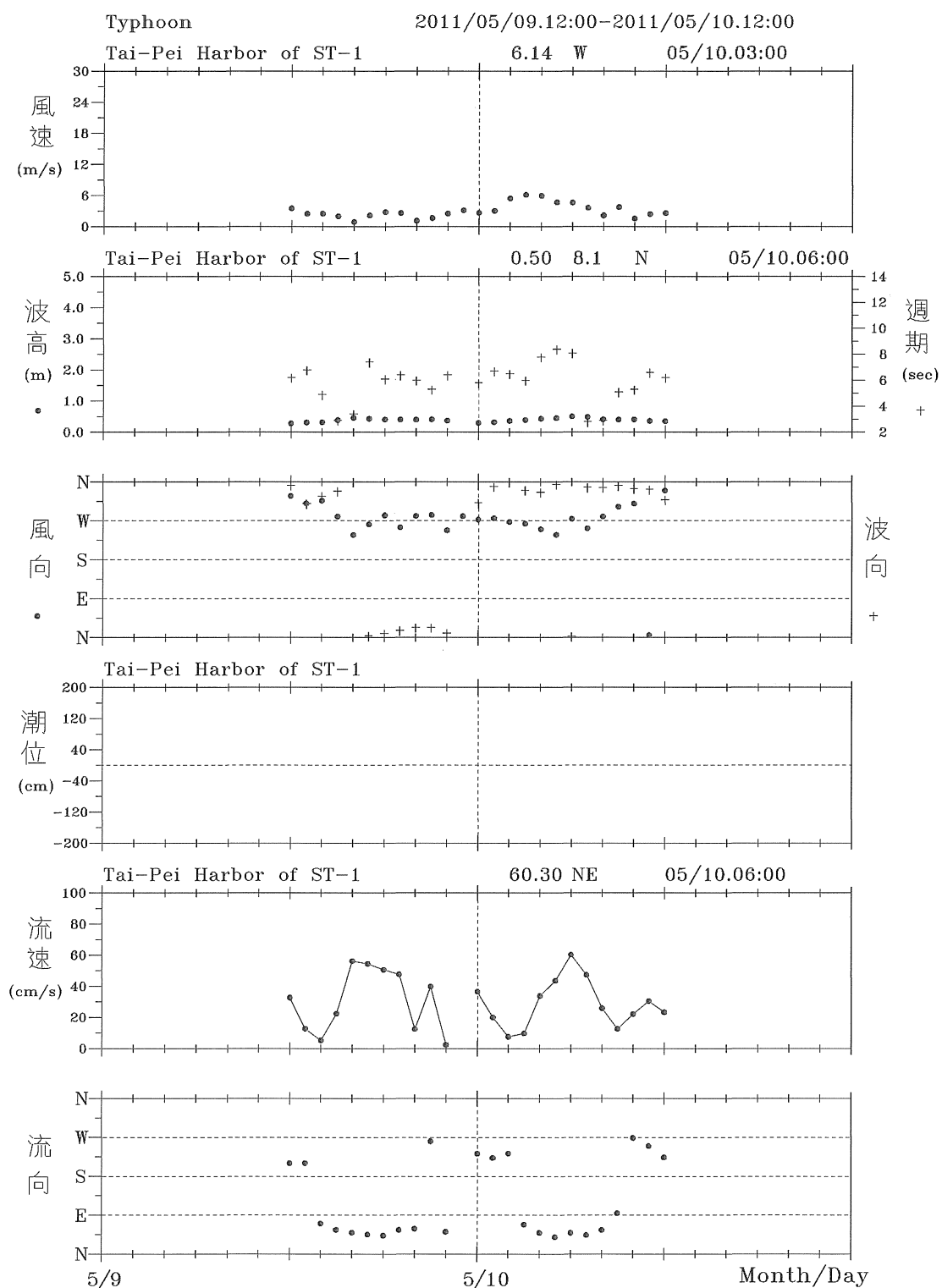
圖 6.3.1 2011 年 5 月艾利颱風臺北港風、潮、浪、流歷線圖
