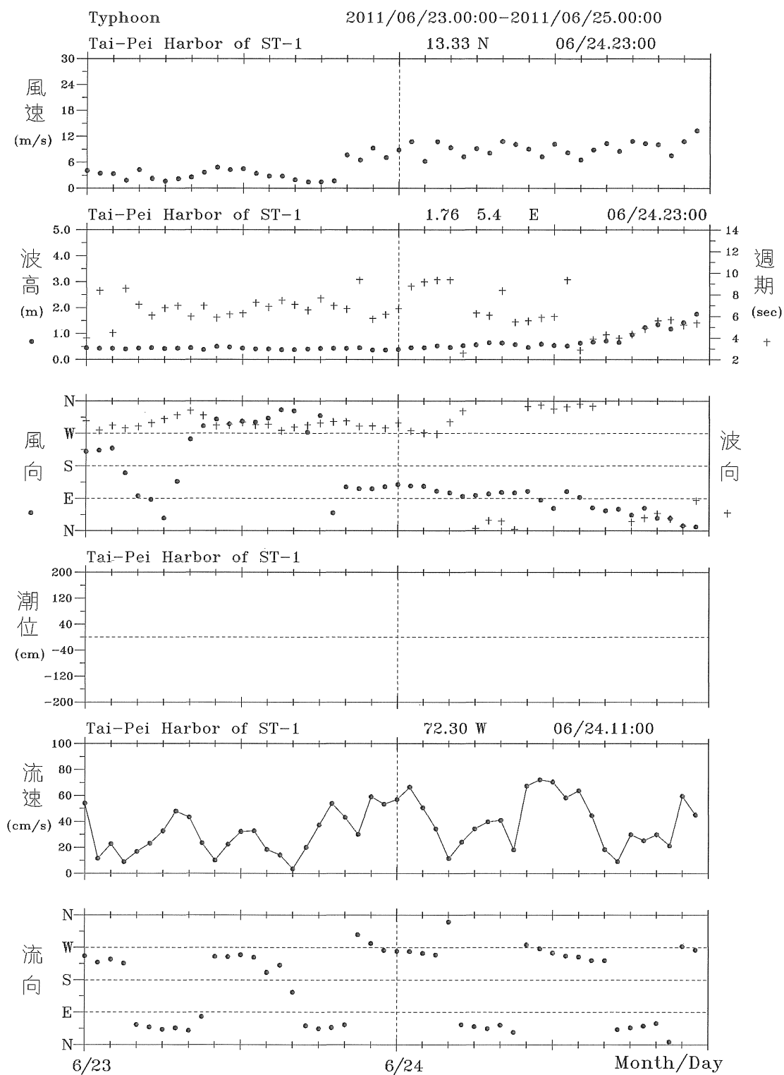
圖6.3.3 2011年6月米雷颱風臺北港風、潮、浪、流歷線圖
