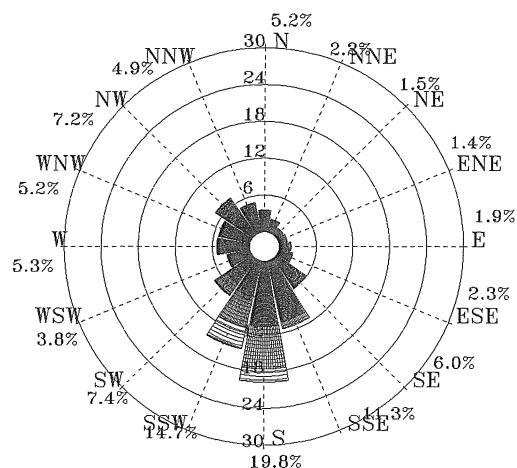
圖 5.2.40 2011 年 3 月馬公港 1 站海流玫瑰圖
