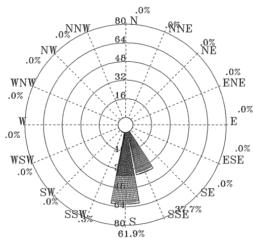
圖 4.2.37 2011 年 1 月馬公港 1 站波浪玫瑰圖
