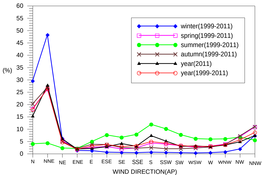
圖 3.4.b 安平港歷年四季及 2011 年、歷年全期風向機率分佈圖
