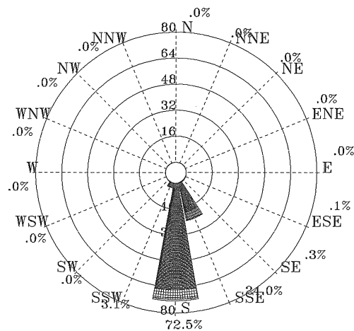
圖 4.2.41 2011 年 4 月馬公港 1 站波浪玫瑰圖
