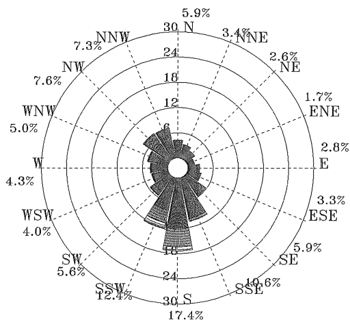
圖 5.2.43 2011 年春季馬公港 1 站海流玫瑰圖
