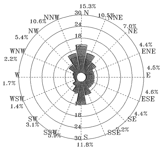
圖 5.2.47 2011 年夏季馬公港 1 站海流玫瑰圖
