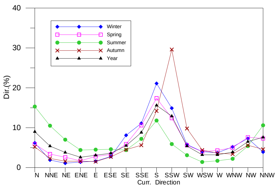
圖 5.5.c 馬公港 2011 年四季及全年海流流向分佈比率圖
