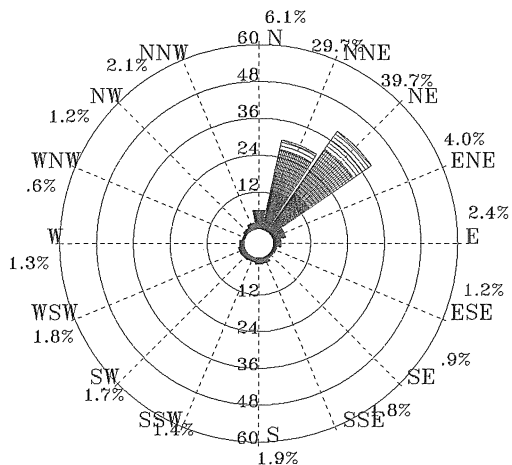
圖 3.2.44 歷年春季馬公港 1 站風玫瑰圖
