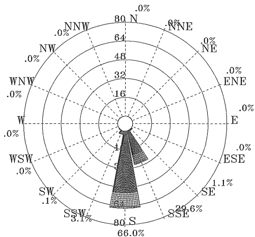
圖 4.2.42 2011 年 5 月馬公港 1 站波浪玫瑰圖
