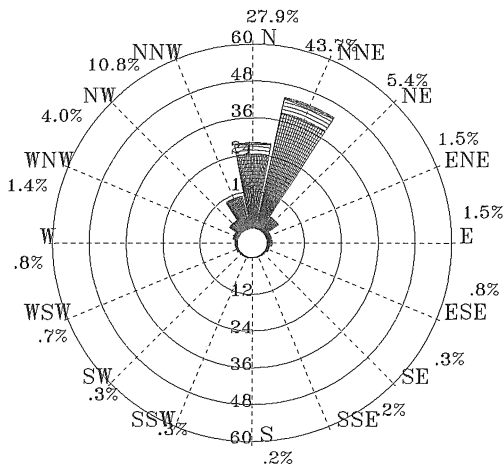
圖 3.2.33 歷年 11 月安平港 1 站風玫瑰圖
