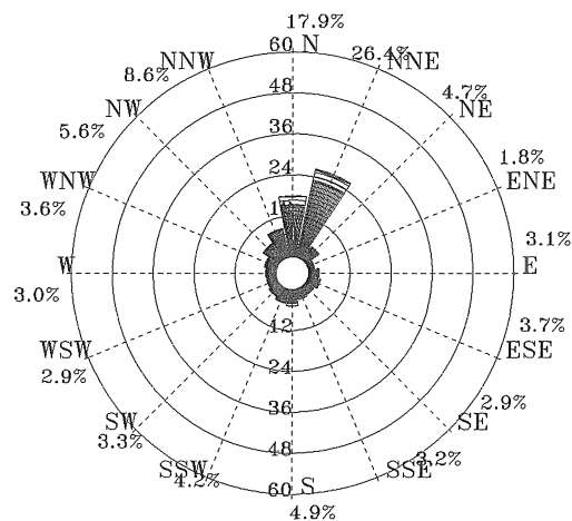
圖 3.2.36 歷年 1999-2011 全年安平港 1 站風玫瑰圖
