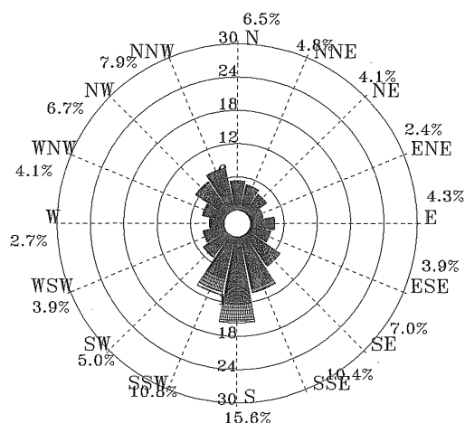
圖 5.2.41 2011 年 4 月馬公港 1 站海流玫瑰圖
