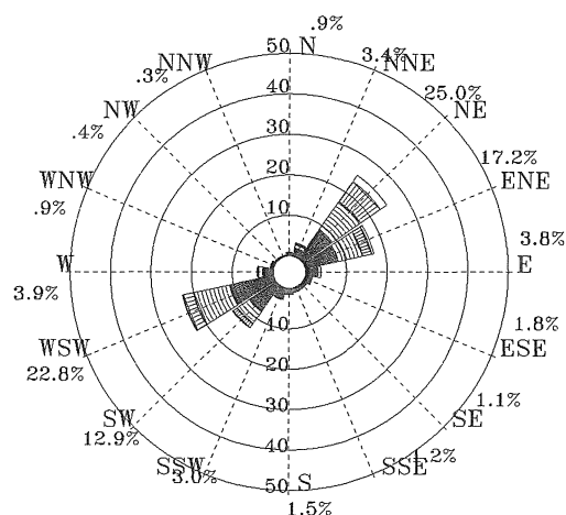
圖 5.2.6 歷年 4 月臺北港 1 站海流玫瑰圖
