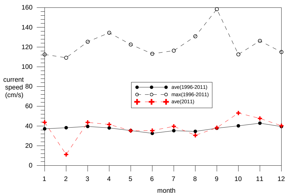
圖 5.6.a 臺北港歷年月平均流速及極值圖
