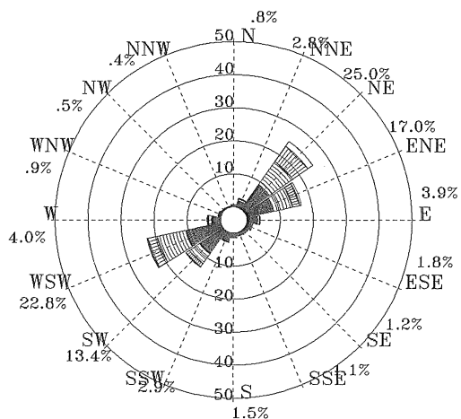
圖 5.2.8 歷年春季臺北港 1 站海流玫瑰圖
