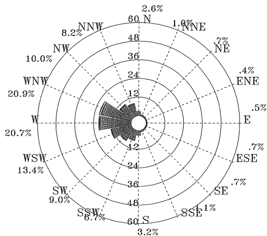
圖 4.2.19 歷年 12 月安平港 1 站波浪玫瑰圖
