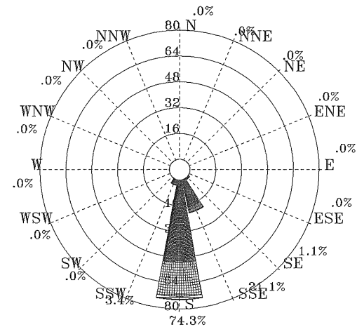
圖 4.2.45 2011 年 7 月馬公港 1 站波浪玫瑰圖
