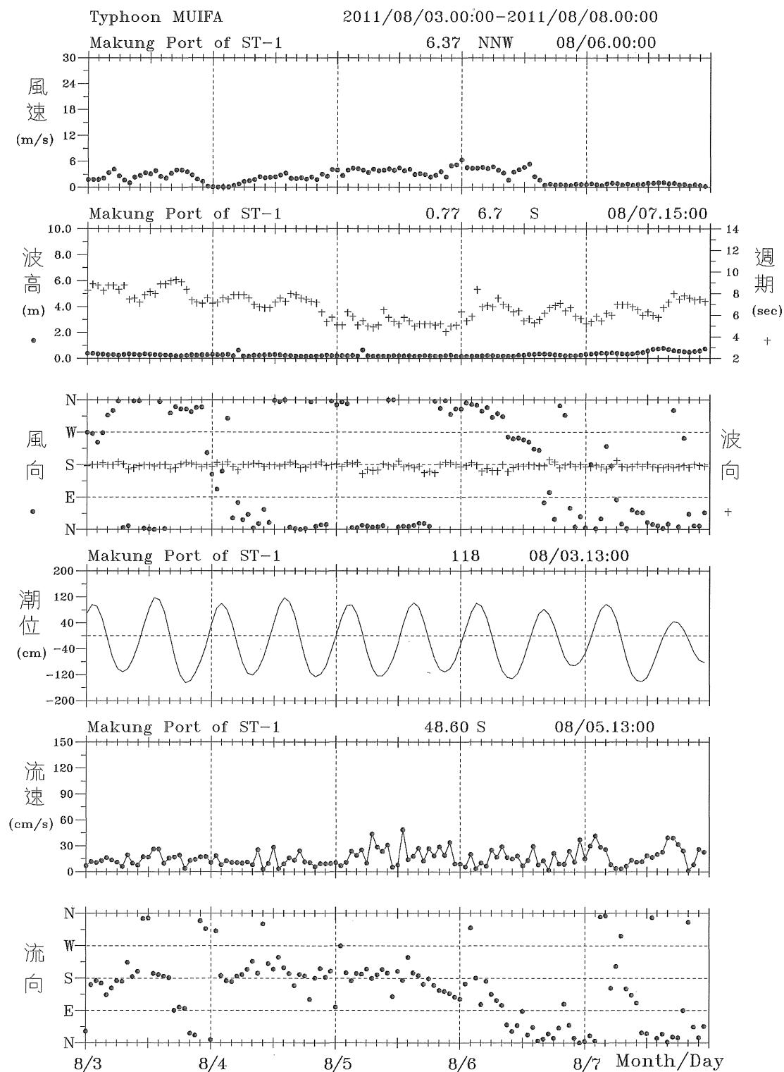
圖 6.3.14 2011 年 8 月梅花颱風馬公港測站風、潮、浪、流歷線圖
