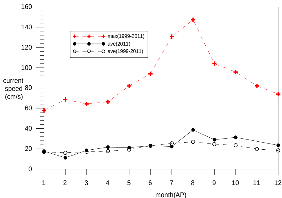
圖 5.6.b 安平港歷年月平均流速及極值圖
