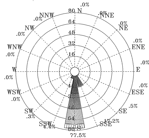
圖 4.2.44 2011 年 6 月馬公港 1 站波浪玫瑰圖
