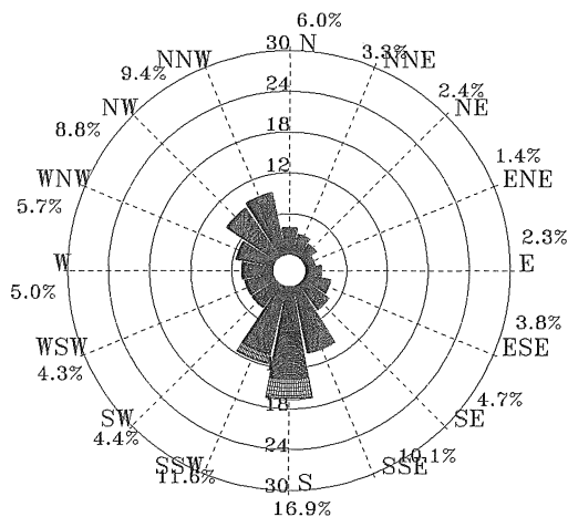
圖 5.2.42 2011 年 5 月馬公港 1 站海流玫瑰圖
