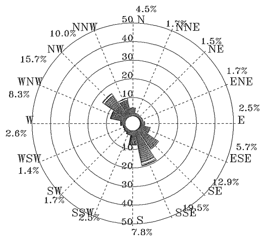
圖 5.2.25 歷年 5 月安平港 1 站海流玫瑰圖
