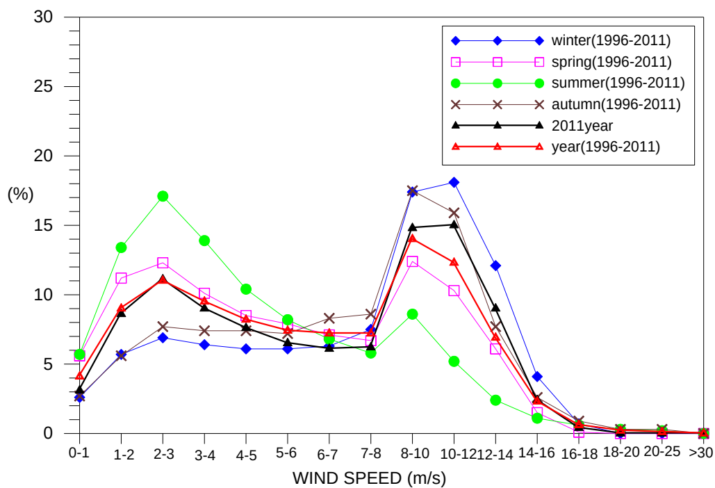
圖 3.3.a 臺北港歷年四季及 2011 年、歷年全期風速機率分佈圖
