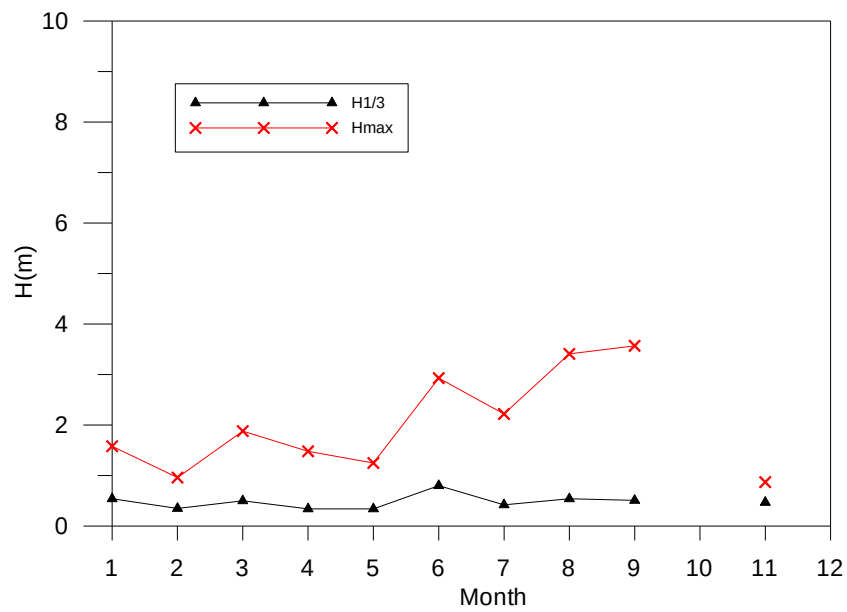
圖 4.6.c 馬公港 2011 年月平均 H_s 波高及 H_s 月極值圖
