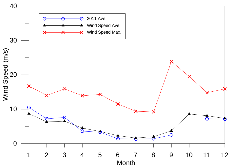
圖 3.6.c 馬公港歷年月平均風速、逐時平均風速月極值變化圖
