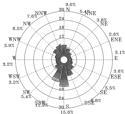
圖 5.2.51 2011 年全年馬公港 1 站海流玫瑰圖
