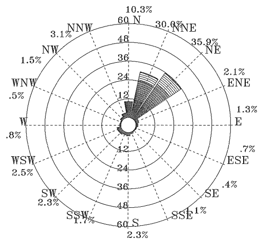
圖 3.2.53 2011 年全年馬公港 1 站風玫瑰圖
