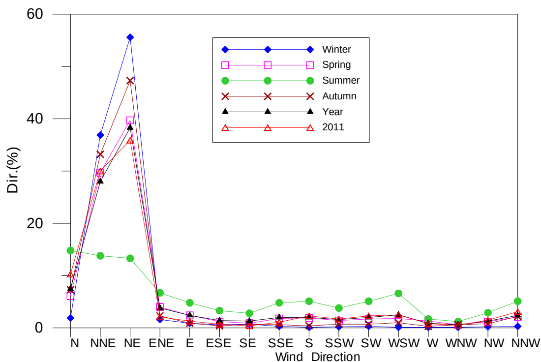
圖 3.4.c 馬公港歷年四季及 2011 年、歷年全期風向機率分佈圖
