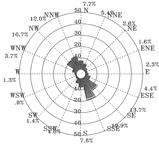
圖 5.2.19 歷年 12 月安平港 1 站海流玫瑰圖
