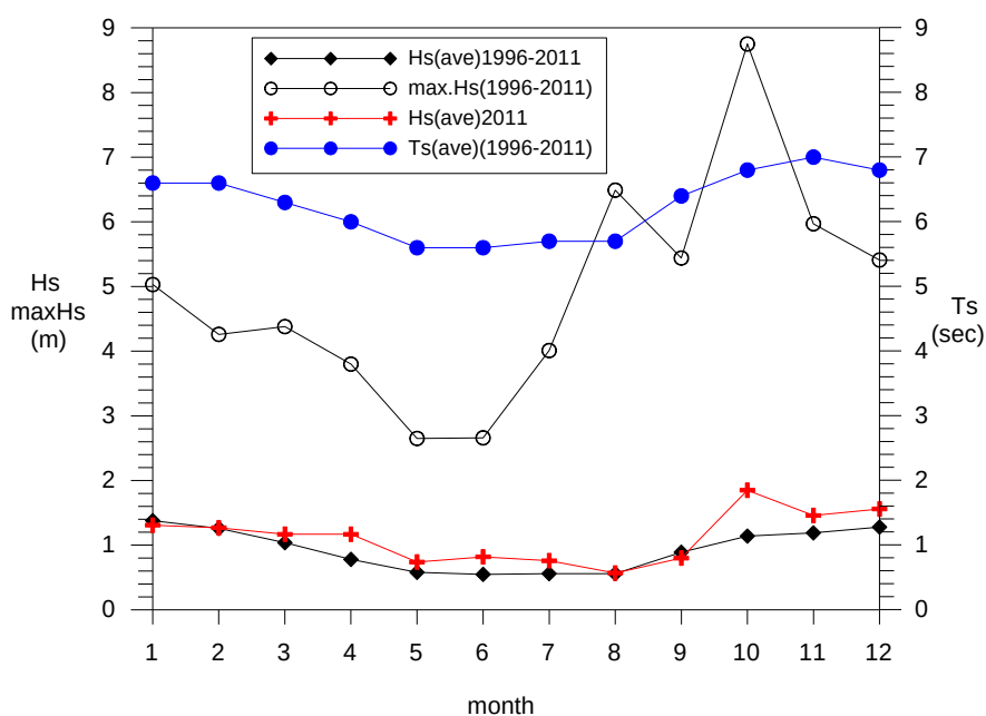
圖 4.6.a 臺北港歷年月平均 H_s 波高及 H_s 月極值圖
