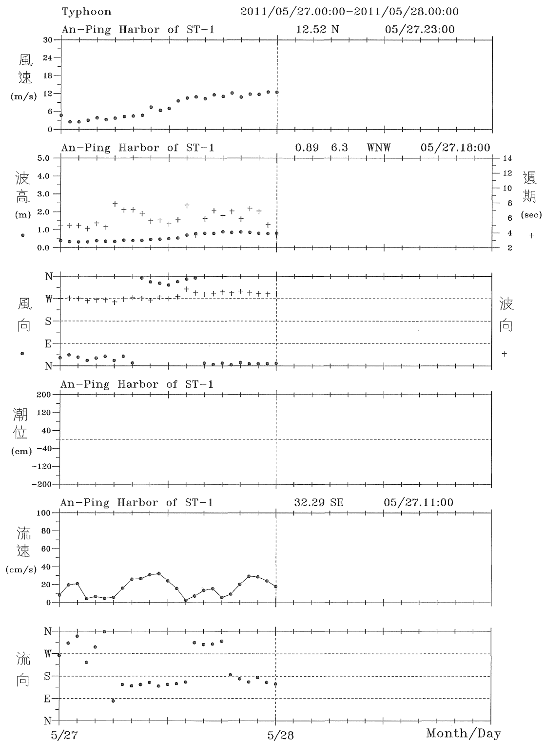
圖 6.3.7 2011 年 5 月桑達颱風安平港風、潮、浪、流歷線圖
