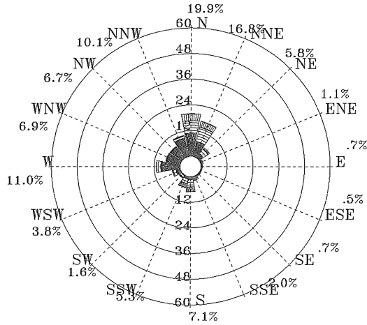
圖 4.2.17 2011 年全年臺北港 1 站波浪玫瑰圖
