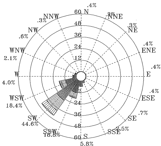
圖 4.2.29 歷年 8 月安平港 1 站波浪玫瑰圖
