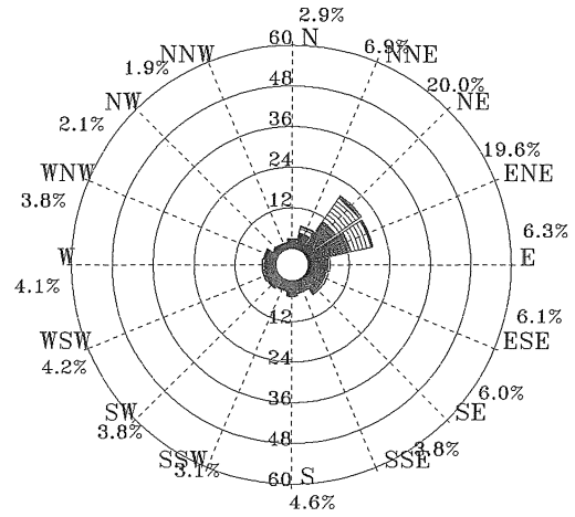
圖 3.2.18 歷年 1996/07/01-2011/11/30 臺北港 1 站風玫瑰圖
