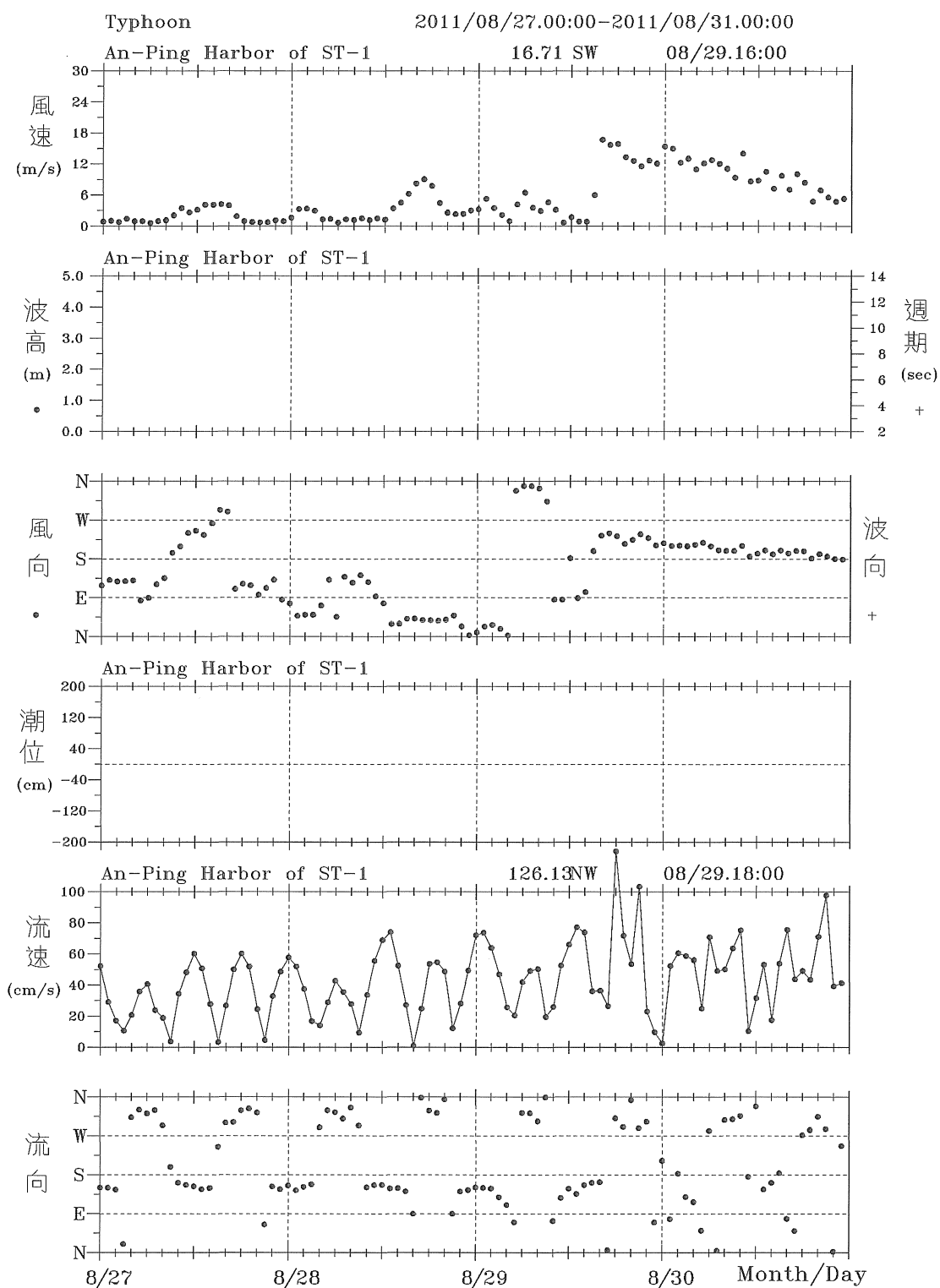
圖 6.3.10 2011 年 8 月南瑪都颱風安平港風、潮、浪、流歷線圖
