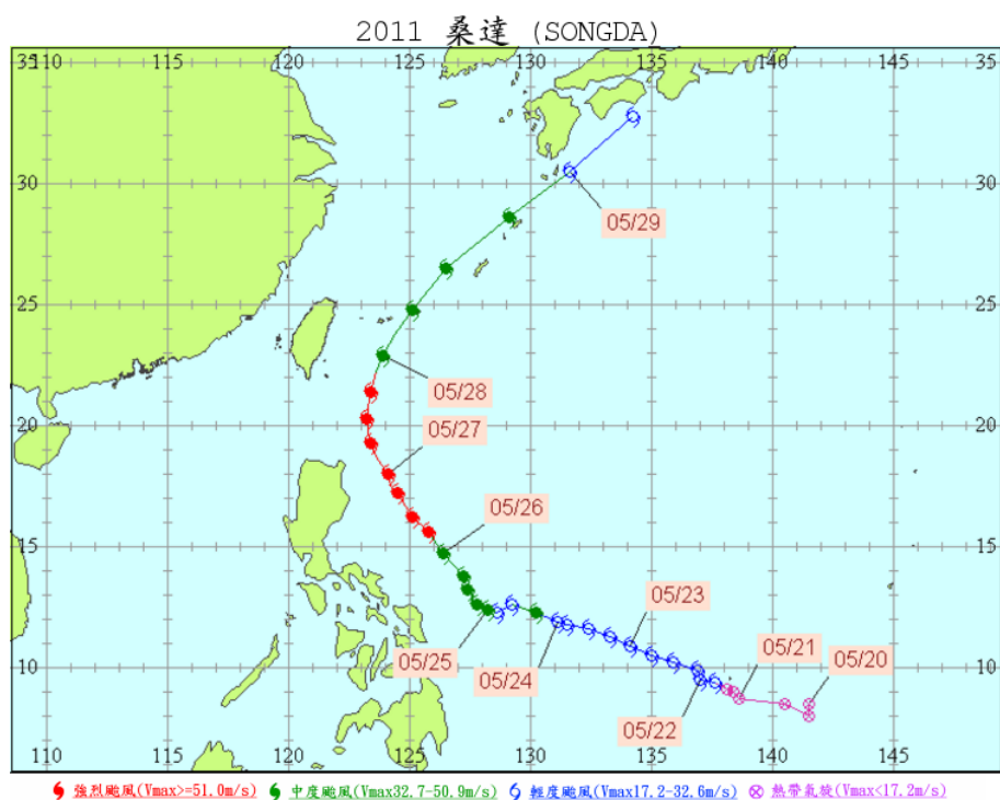
圖 6.2.2 桑達強烈颱風路徑圖
