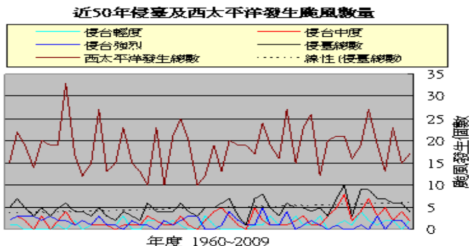
圖 6.1 50 年來西太平洋及侵臺颱風發生頻率圖
