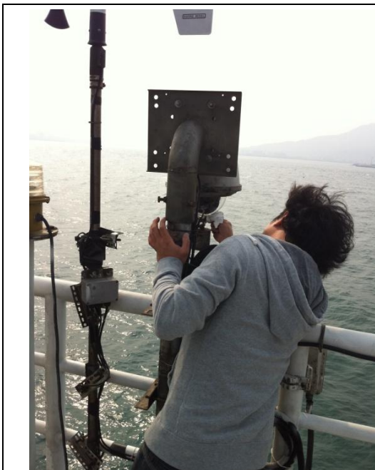
影像監視系統防護罩及雨刷清潔
