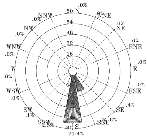
圖 4.2.51 2011 年全年馬公港 1 站波浪玫瑰圖
