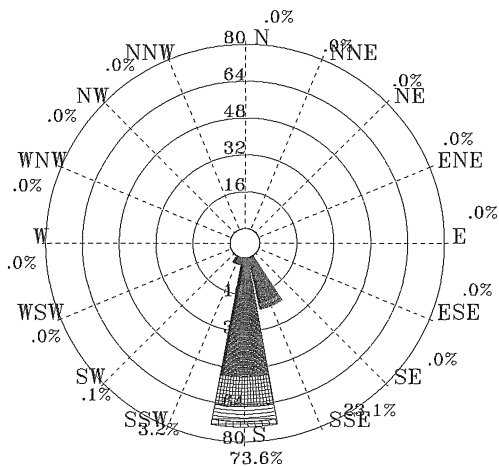
圖 4.2.50 2011 年秋季馬公港 1 站波浪玫瑰圖
