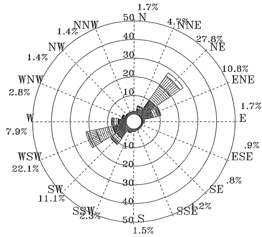
圖 5.2.17 2011 年全年臺北港 1 站海流玫瑰圖
