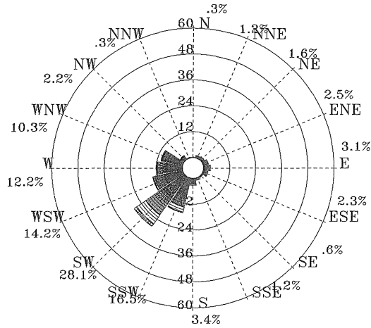
圖 4.2.35 2011 年全年安平港 1 站波浪玫瑰圖
