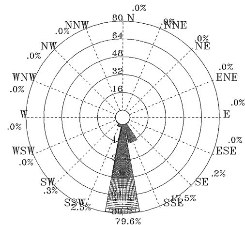
圖 4.2.46 2011 年 8 月馬公港 1 站波浪玫瑰圖
