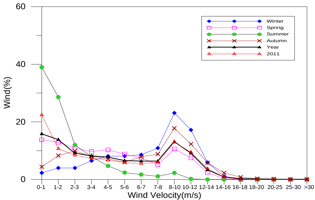
圖 3.3.c 馬公港歷年四季及 2011 年、歷年全期風速機率分佈圖
