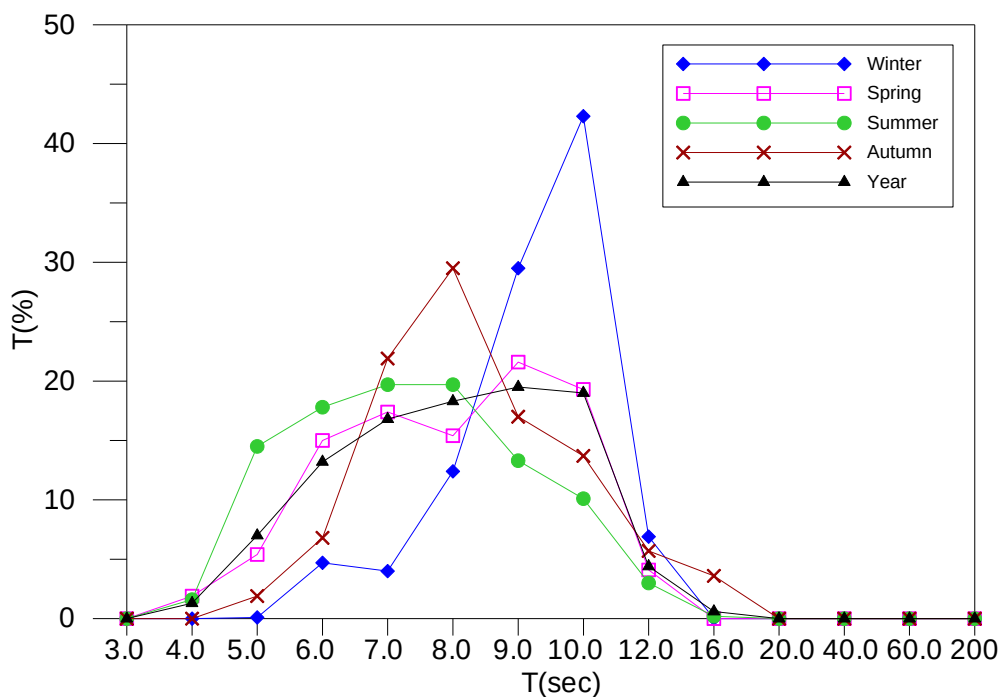
圖 4.4.c 馬公港 2011 年四季及全觀測期波浪週期機率分佈圖
