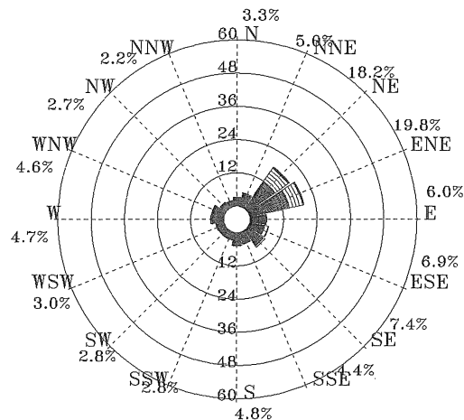
圖 3.2.6 歷年 4 月臺北港 1 站風玫瑰圖
