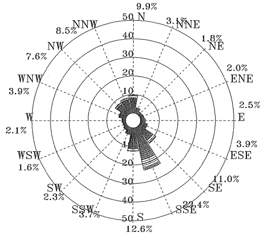
圖 5.2.35 2011年全年安平港1站海流玫瑰圖
