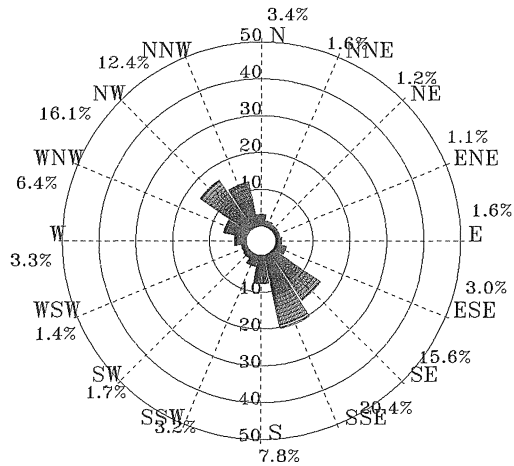
圖 5.2.21 歷年 2 月安平港 1 站海流玫瑰圖
