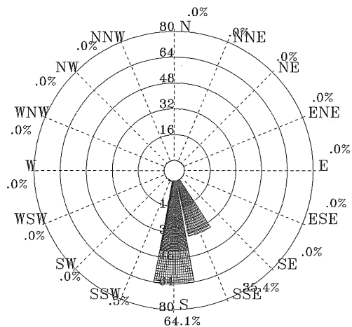
圖 4.2.39 2011 年冬季馬公港 1 站波浪玫瑰圖
