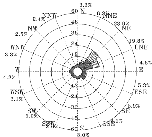
圖 3.2.5 歷年 3 月臺北港 1 站風玫瑰圖
