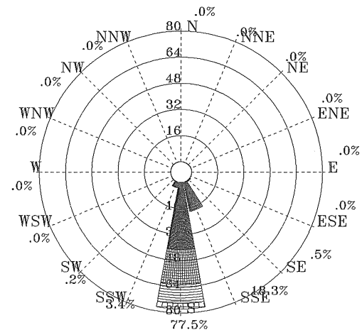
圖 4.2.47 2011 年夏季馬公港 1 站波浪玫瑰圖
