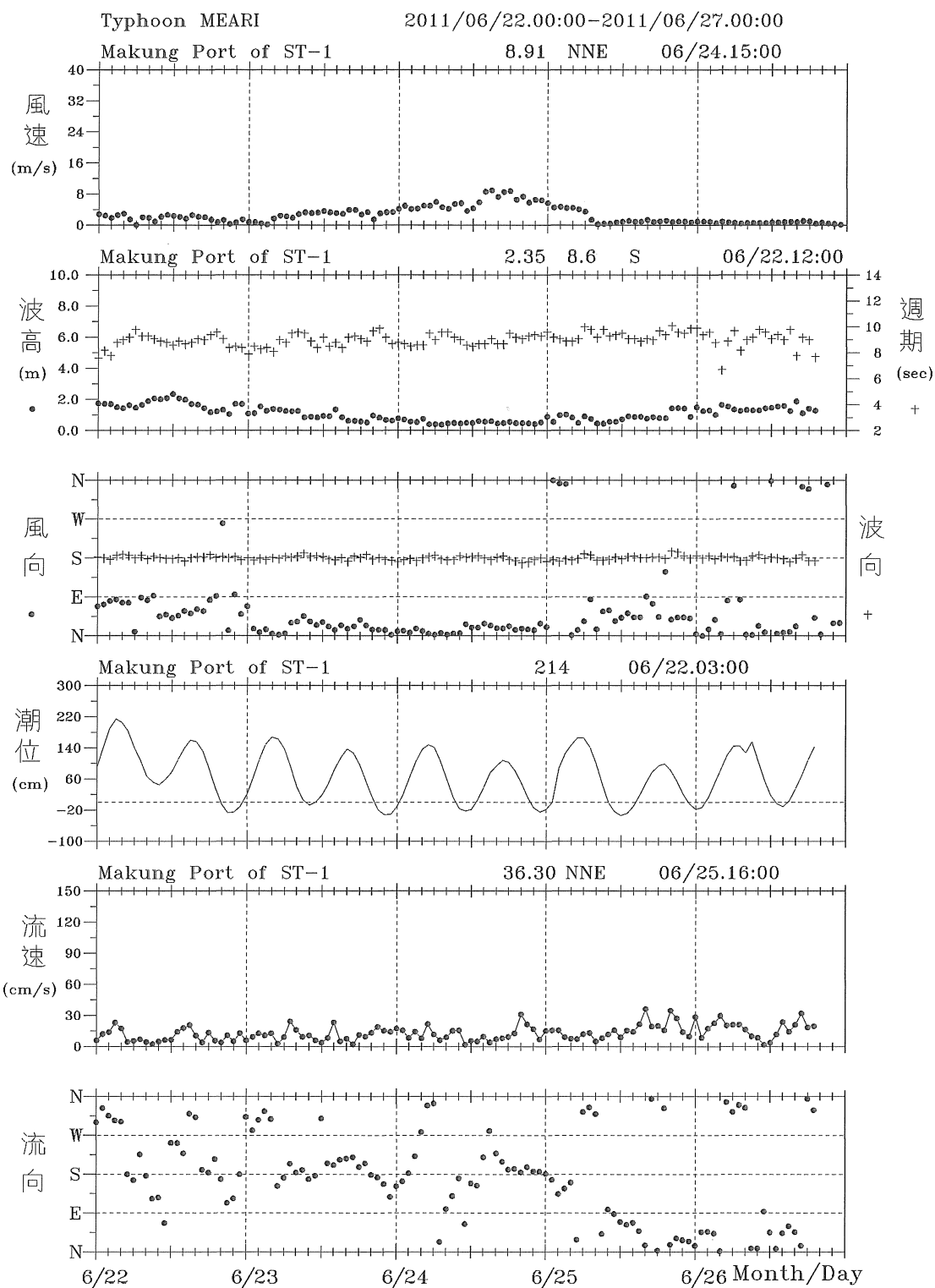
圖 6.3.13 2011 年 6 月米雷颱風馬公港測站風、潮、浪、流歷線圖
