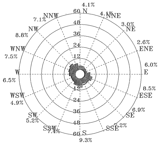
圖 3.2.29 歷年 8 月安平港 1 站風玫瑰圖
