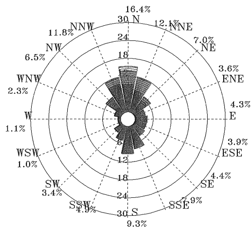
圖 5.2.44 2011 年 6 月馬公港 1 站海流玫瑰圖
