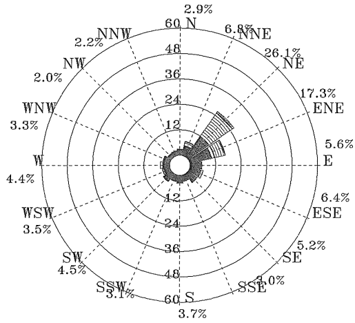
圖 3.2.17 2011 年全年臺北港 1 站風玫瑰圖
