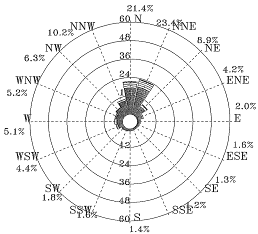
圖 4.2.7 歷年 5 月臺北港 1 站波浪玫瑰圖
