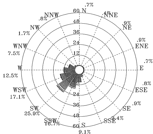
圖 4.2.25 歷年 5 月安平港 1 站波浪玫瑰圖
