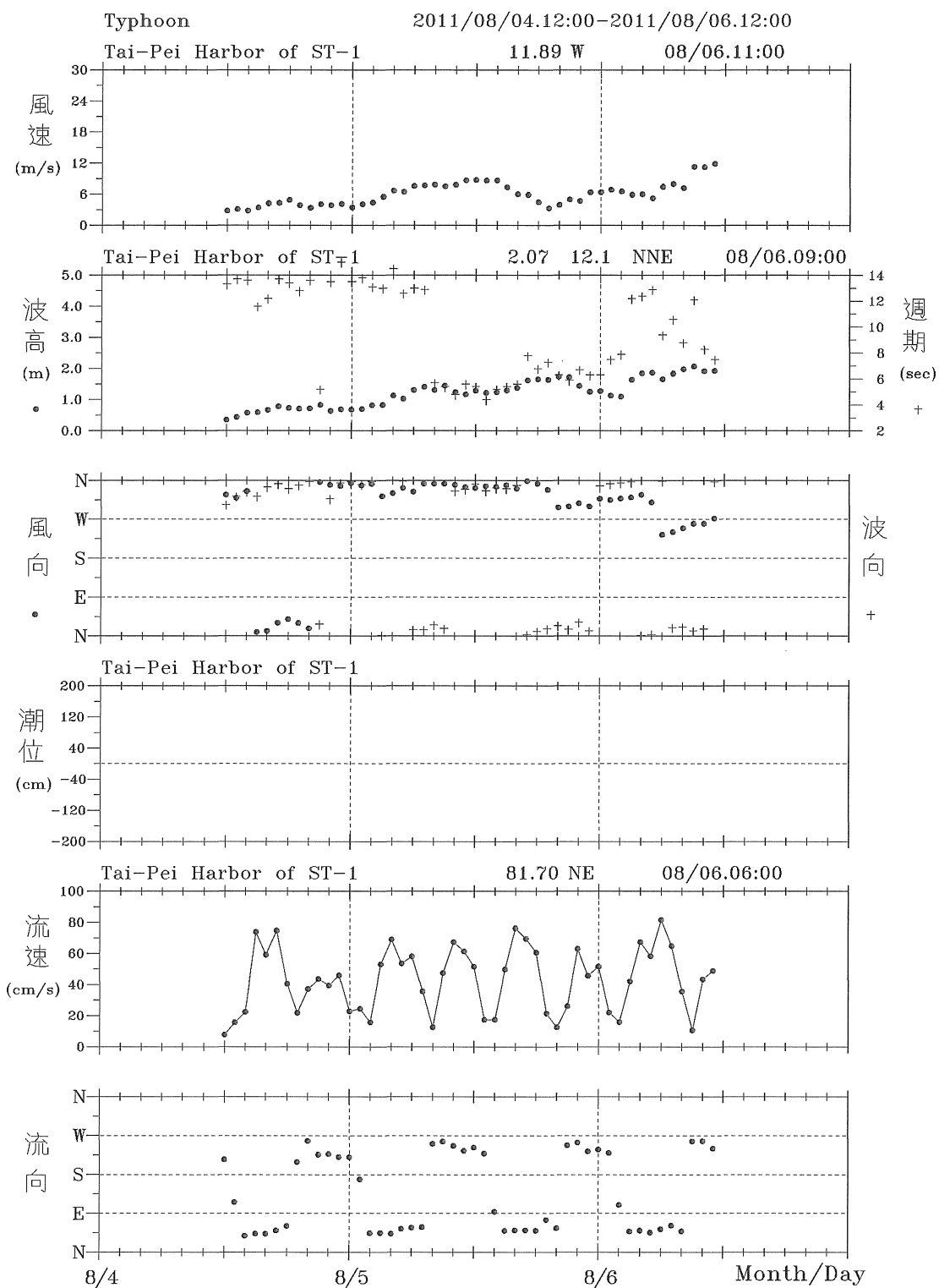
圖 6.3.4 2011 年 8 月梅花颱風臺北港風、潮、浪、流歷線圖
