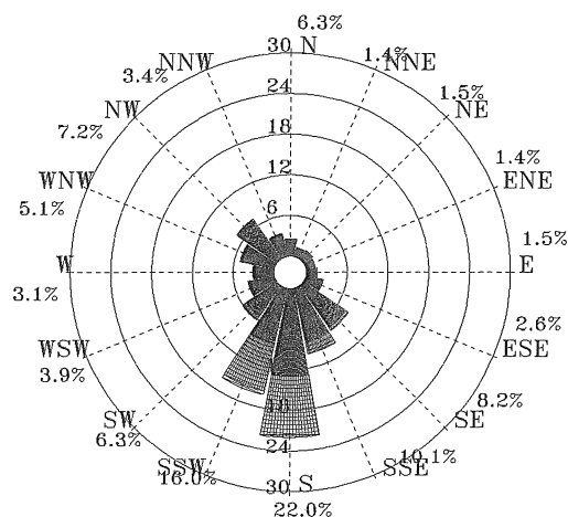
圖 5.2.37 2011 年 1 月馬公港 1 站海流玫瑰圖
