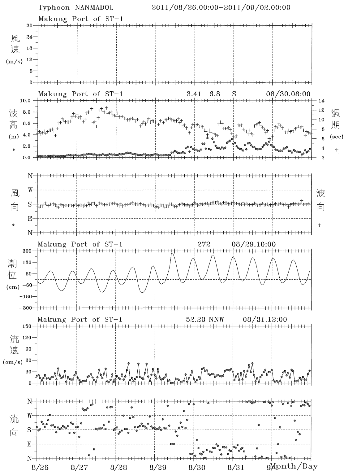
圖 6.3.15 2011 年 8 月南瑪都颱風馬公港測站風、潮、浪、流歷線圖
