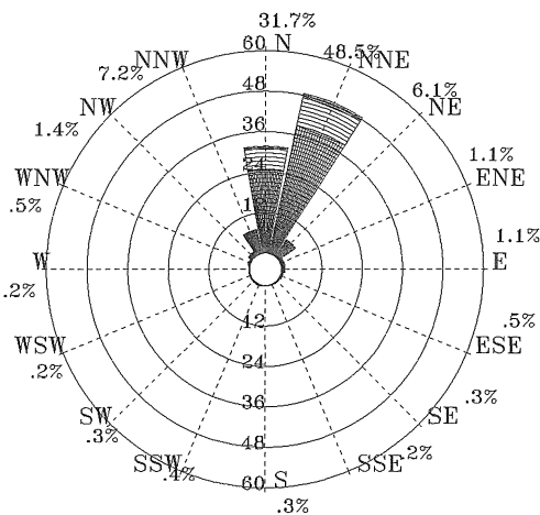
圖 3.2.20 歷年 1 月安平港 1 站風玫瑰圖
