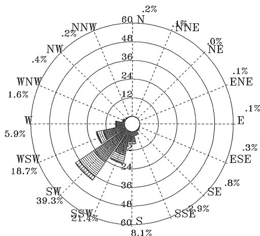
圖 4.2.27 歷年 6 月安平港 1 站波浪玫瑰圖
