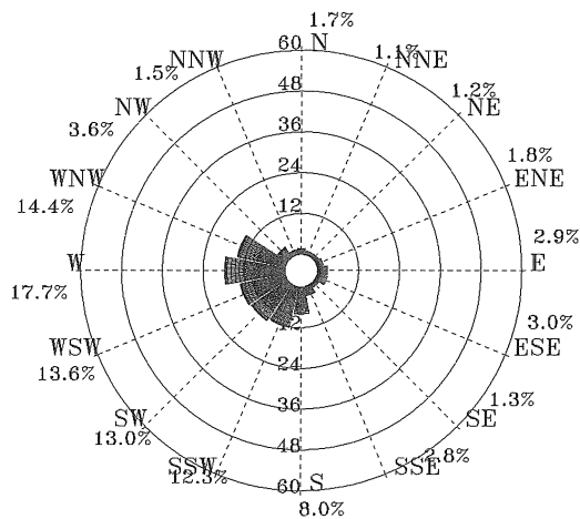
圖 4.2.24 歷年 4 月安平港 1 站波浪玫瑰圖
