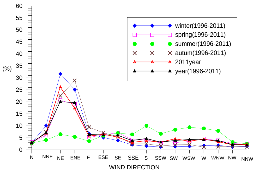
圖 3.4.a 臺北港歷年四季及 2011 年、歷年全期風向機率分佈圖
