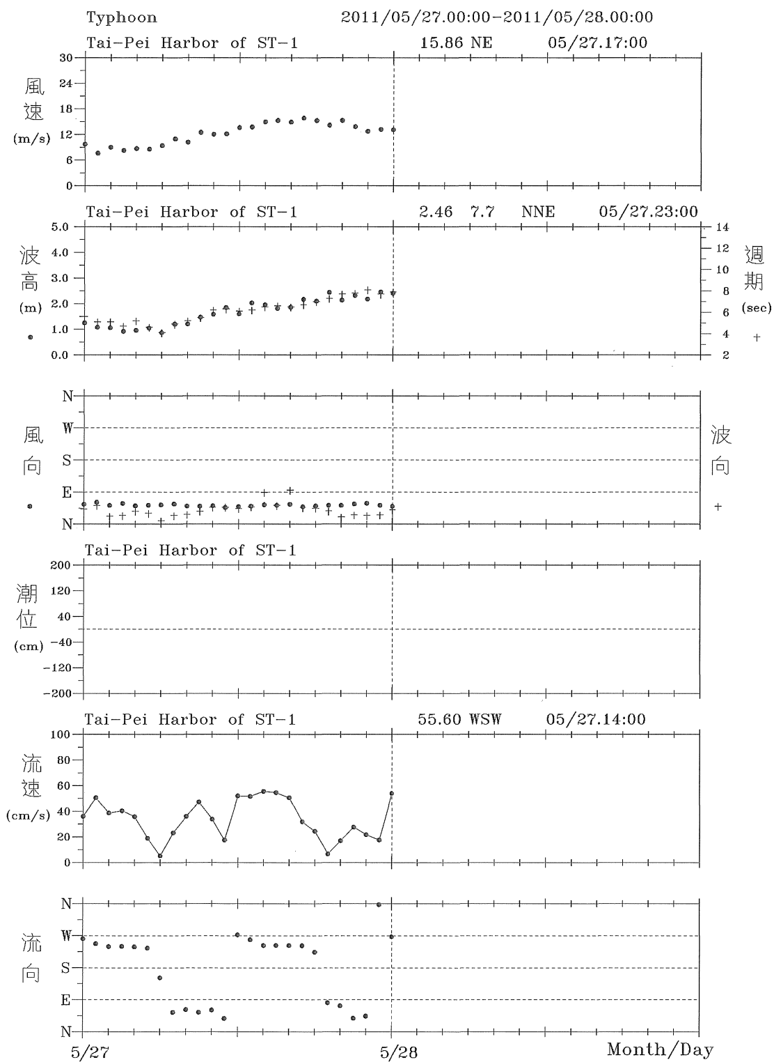
圖 6.3.2 2011 年 5 月桑達颱風臺北港風、潮、浪、流歷線圖
