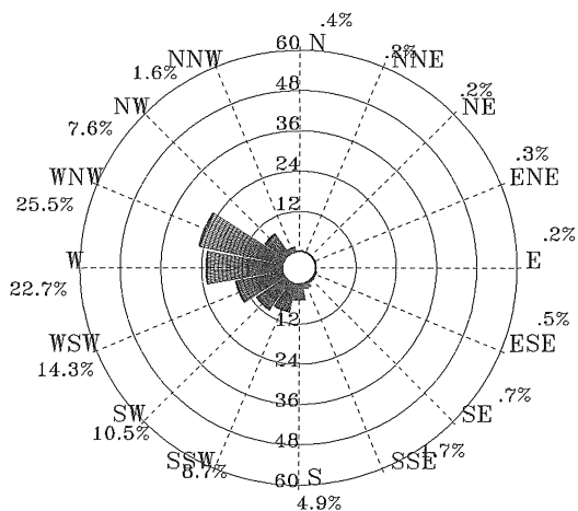
圖 4.2.33 歷年 11 月安平港 1 站波浪玫瑰圖
