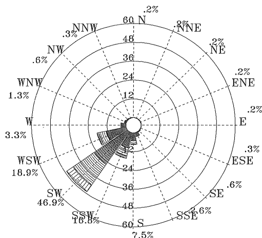
圖 4.2.28 歷年 7 月安平港 1 站波浪玫瑰圖
