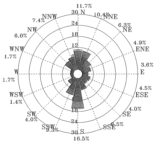
圖 5.2.46 2011 年 8 月馬公港 1 站海流玫瑰圖
