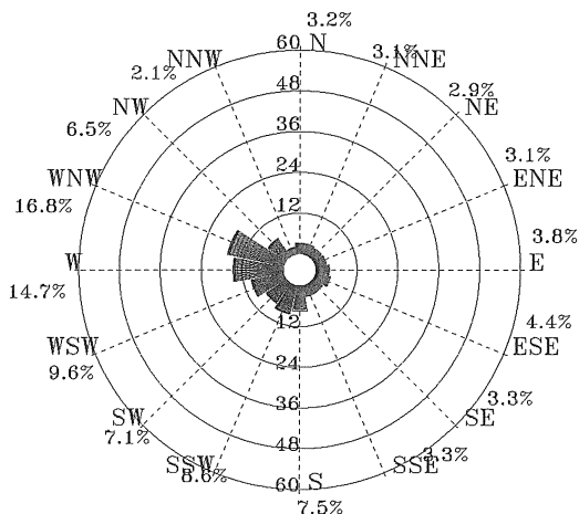
圖 4.2.21 歷年 2 月安平港 1 站波浪玫瑰圖
