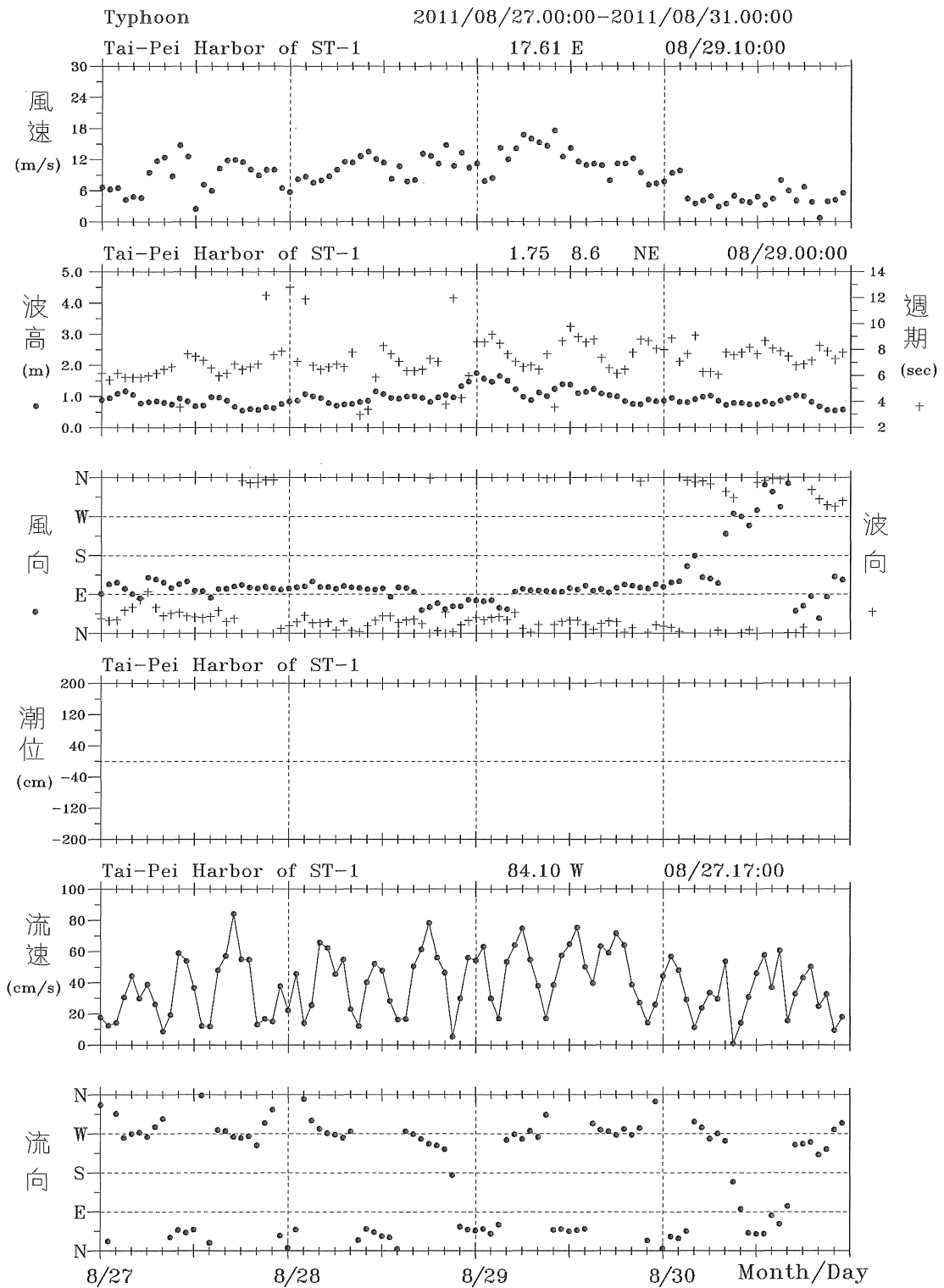
圖6.3.5 2011年8月南瑪都颱風臺北港風、潮、浪、流歷線圖
