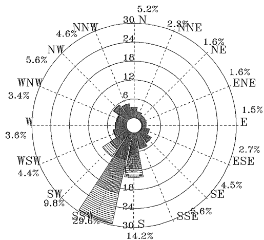
圖 5.2.50 2011 年秋季馬公港 1 站海流玫瑰圖
