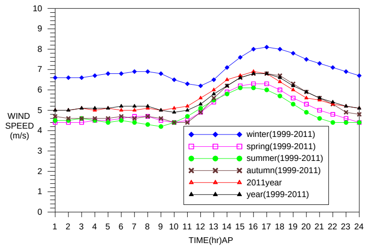
圖 3.5.b 安平港歷年四季日逐時風速變化圖
