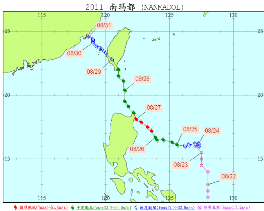
圖 6.2.5 南瑪都強烈颱風路徑圖
