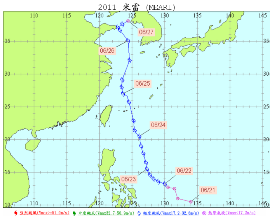
圖 6.2.3 米雷輕度颱風路徑圖
