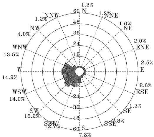
圖 4.2.26 歷年春季安平港 1 站波浪玫瑰圖
