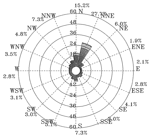
圖 3.2.35 2011 年全年安平港 1 站風玫瑰圖
