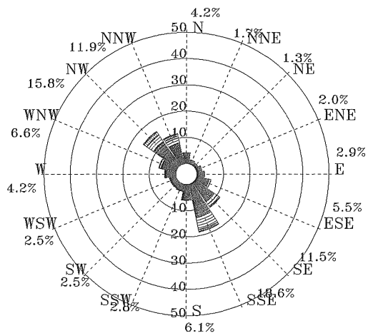
圖 5.2.29 歷年 8 月安平港 1 站海流玫瑰圖
