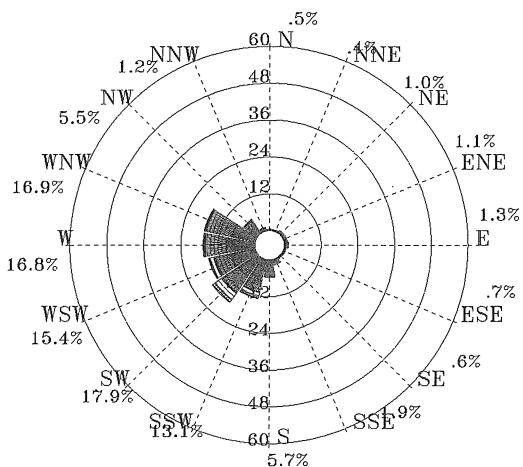
圖 4.2.34 歷年秋季安平港 1 站波浪玫瑰圖
