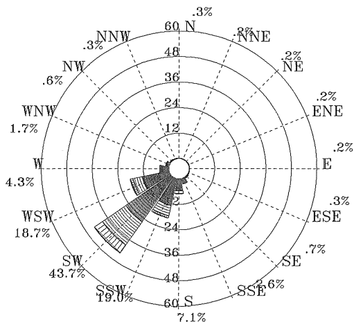
圖 4.2.30 歷年夏季安平港 1 站波浪玫瑰圖
