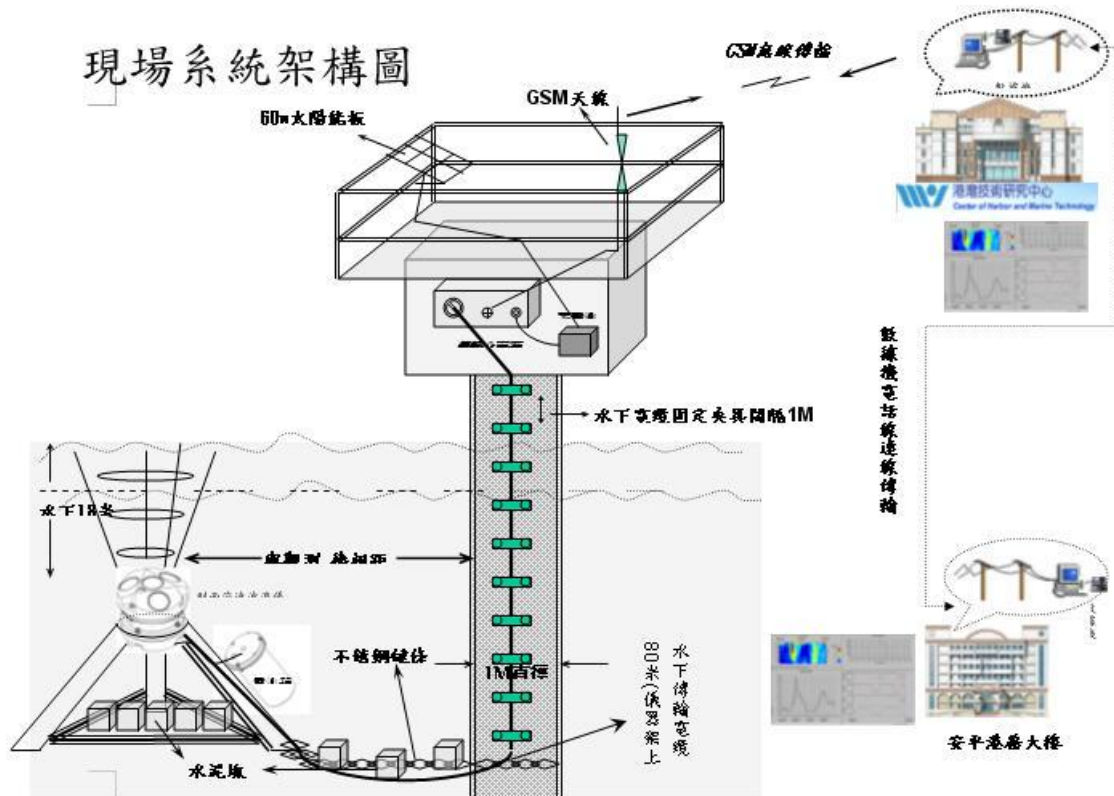
圖 2.9 AWAC 海象觀測系統設計流程
