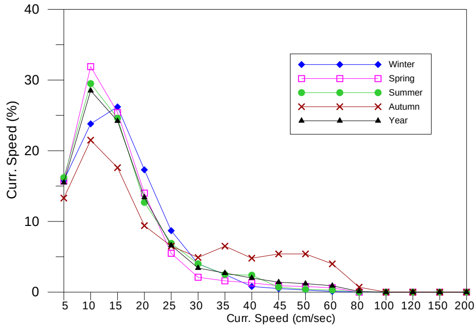
圖 5.4.c 馬公港 2011 年四季及全年海流流速分佈比率圖
