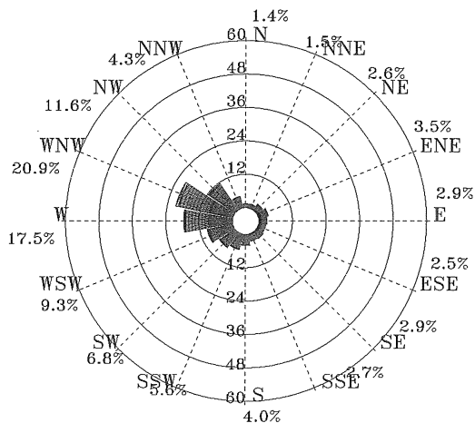
圖 4.2.20 歷年 1 月安平港 1 站波浪玫瑰圖
