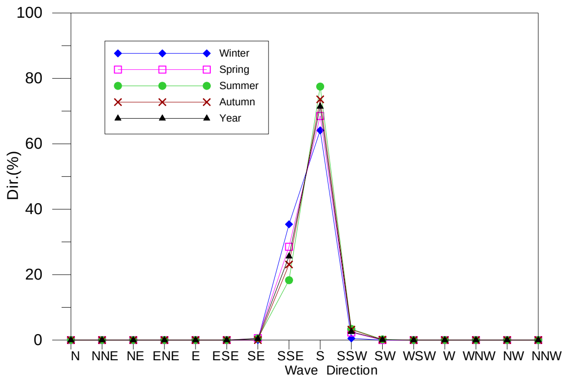
圖 4.5.c 馬公港 2011 年四季及全觀測期波向機率分佈圖
