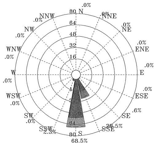
圖 4.2.43 2011 年春季馬公港 1 站波浪玫瑰圖
