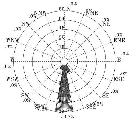
圖 4.2.49 2011 年 11 月馬公港 1 站波浪玫瑰圖
