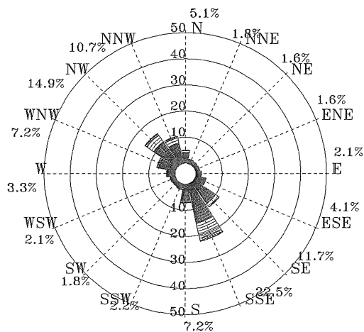
圖 5.2.28 歷年 7 月安平港 1 站海流玫瑰圖
