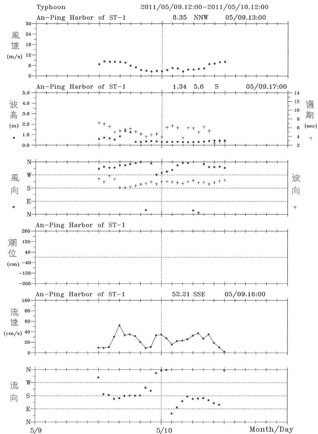
圖 6.3.6 2011 年 5 月艾利颱風安平港風、潮、浪、流歷線圖
