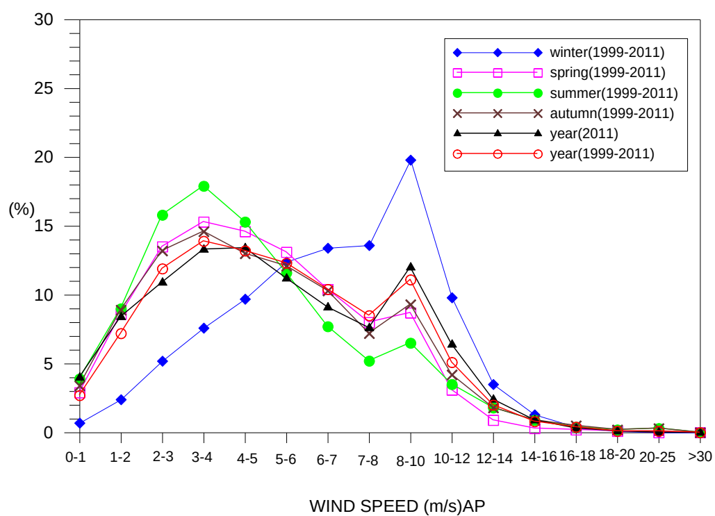
圖 3.3.b 安平港歷年四季及 2011 年、歷年全期風速機率分佈圖
