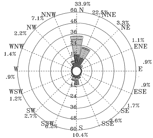
圖 4.2.14 歷年 10 月臺北港 1 站波浪玫瑰圖
