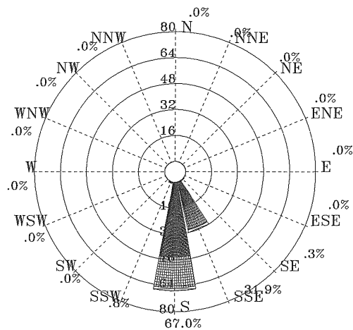
圖 4.2.40 2011 年 3 月馬公港 1 站波浪玫瑰圖
