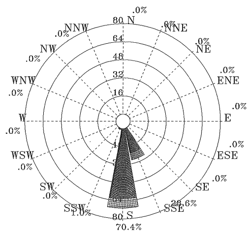
圖 4.2.38 2011 年 2 月馬公港 1 站波浪玫瑰圖
