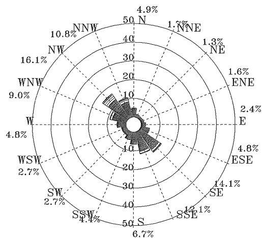
圖 5.2.27 歷年 6 月安平港 1 站海流玫瑰圖
