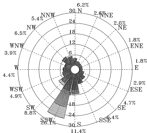
圖 5.2.48 2011 年 9 月馬公港 1 站海流玫瑰圖
