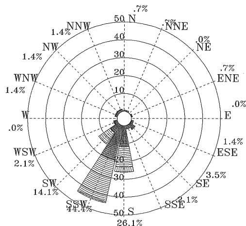
圖 5.2.49 2011 年 11 月馬公港 1 站海流玫瑰圖
