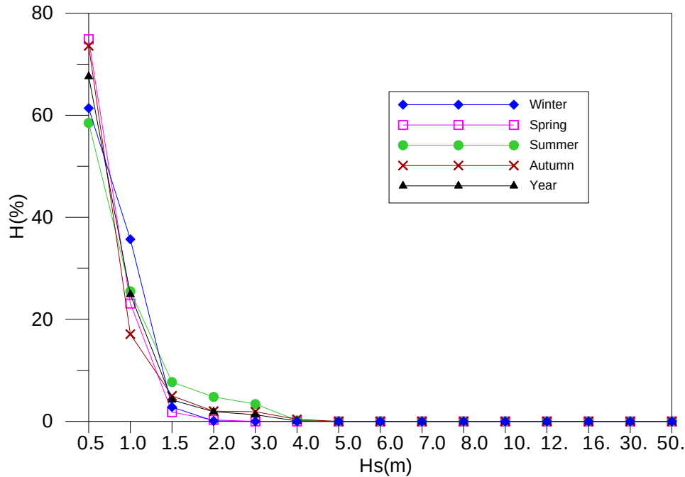
圖 4.3.c 馬公港 2011 年四季及全觀測期波高機率分佈圖
