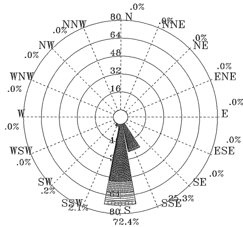
圖 4.2.48 2011 年 9 月馬公港 1 站波浪玫瑰圖
