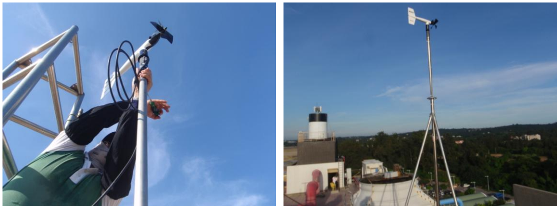
圖 2.7 氣象觀測用 Yang 風速風向計儀器
