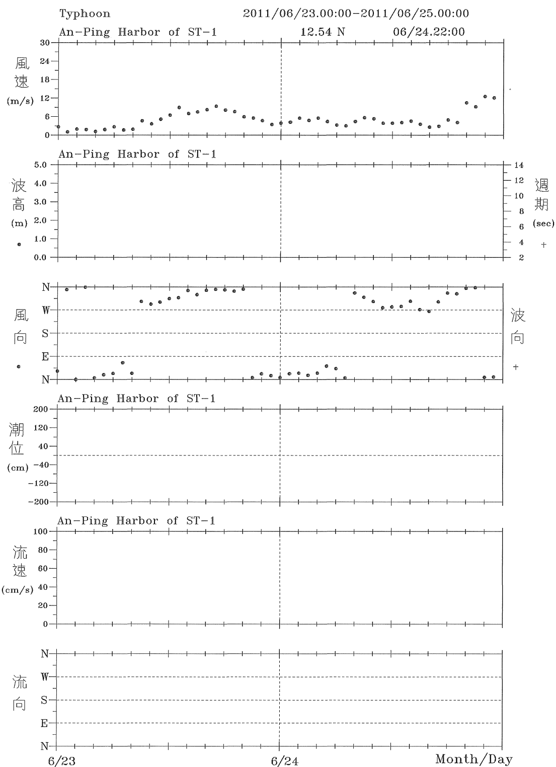
圖 6.3.8 2011 年 6 月米雷颱風安平港風、潮、浪、流歷線圖
