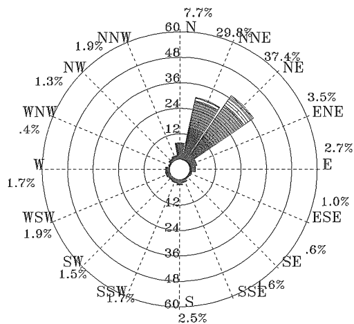
圖 3.2.42 歷年 4 月馬公港 1 站風玫瑰圖
