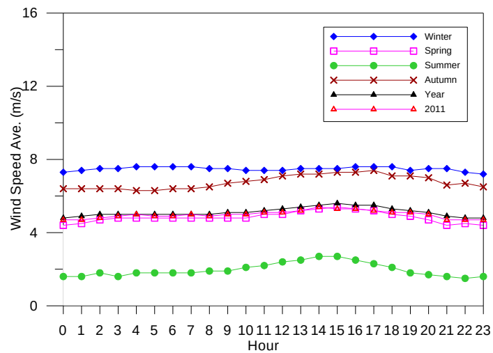
圖 3.5.c 馬公港歷年四季四季日逐時風速變化圖
