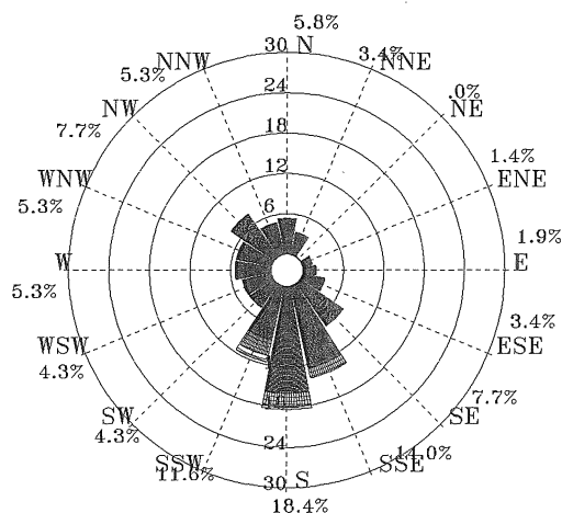
圖 5.2.38 2011 年 2 月馬公港 1 站海流玫瑰圖
