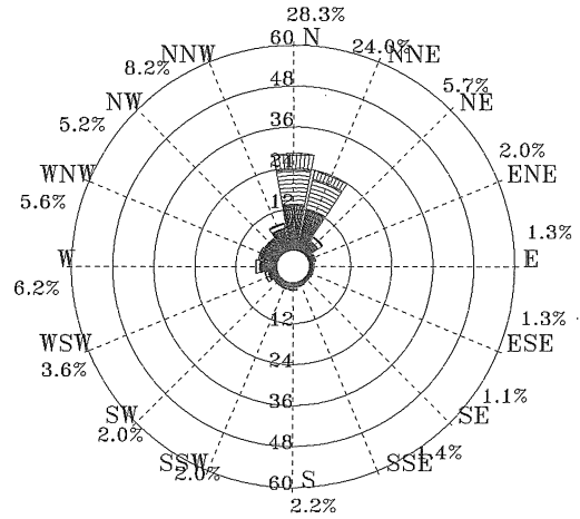
圖 4.2.18 歷年 1996/07/01-2011/11/30 全年臺北港 1 站波浪玫瑰圖
