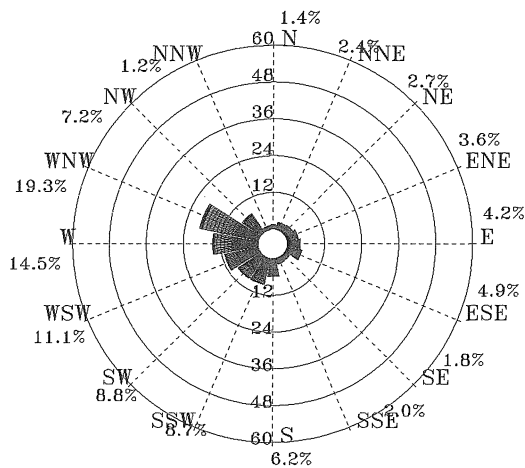
圖 4.2.23 歷年 3 月安平港 1 站波浪玫瑰圖
