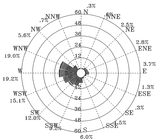
圖 4.2.32 歷年 10 月安平港 1 站波浪玫瑰圖
