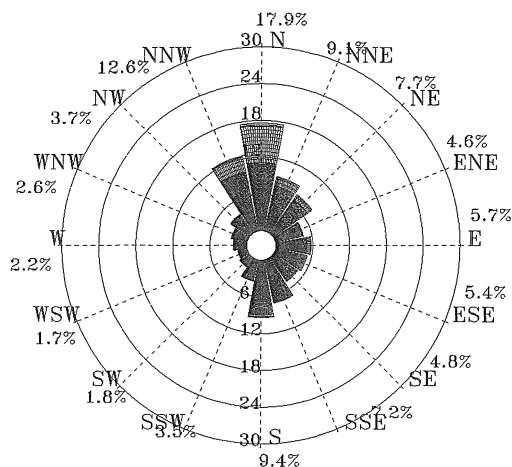
圖 5.2.45 2011 年 7 月馬公港 1 站海流玫瑰圖
