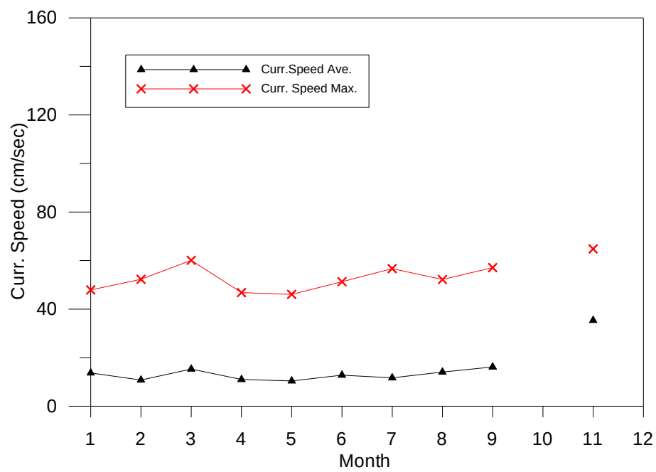
圖 5.6.c 馬公港 2011 年月平均流速及極值圖
