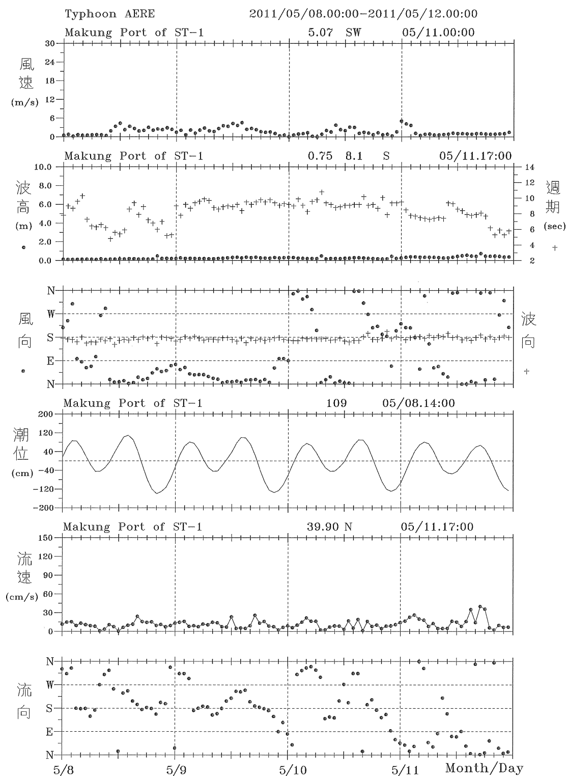
圖 6.3.11 2011 年 5 月艾利颱風馬公港測站風、潮、浪、流歷線圖
