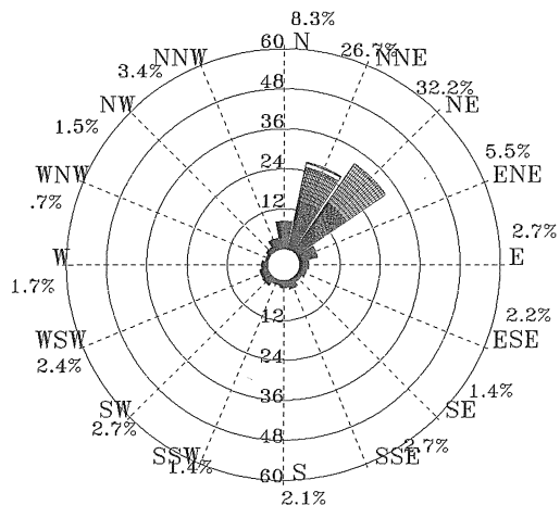
圖 3.2.43 歷年 5 月馬公港 1 站風玫瑰圖
