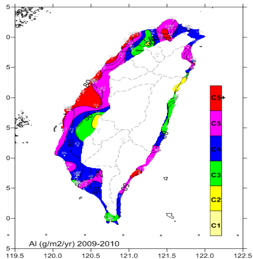
圖 6-28 2009-2010 鋁年腐蝕速率 ISO 分類圖
