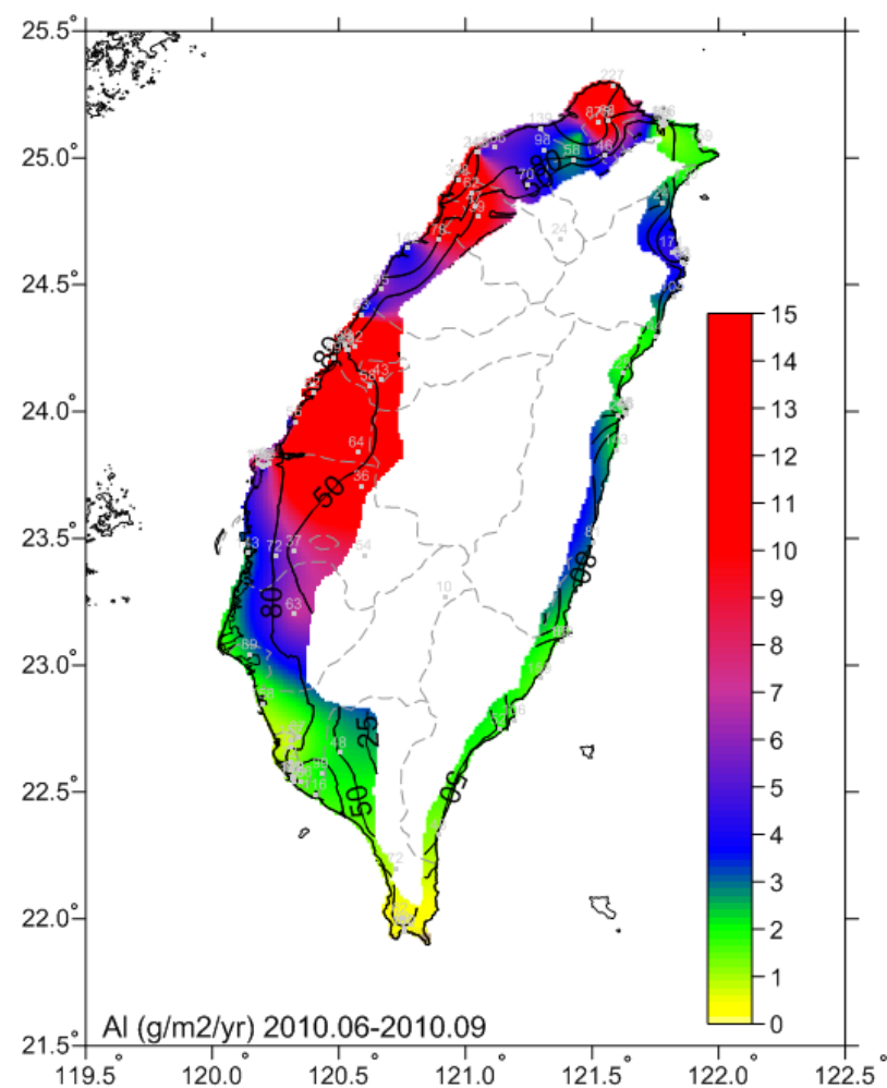
圖 6-24 2010.06-2010.09 鋁腐蝕速率圖
