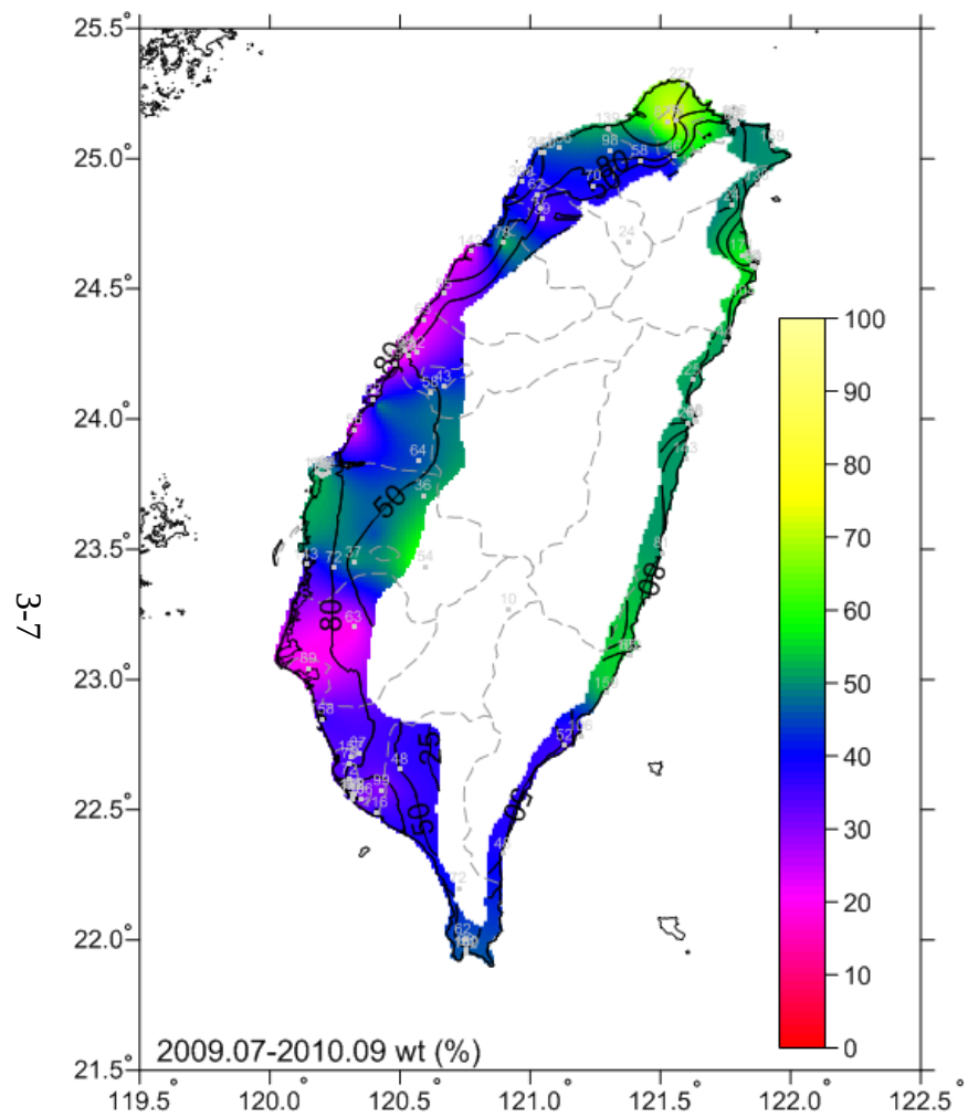
圖 3-5 2009.07-2010.09 一年期濕潤時間(百分比)等位圖
