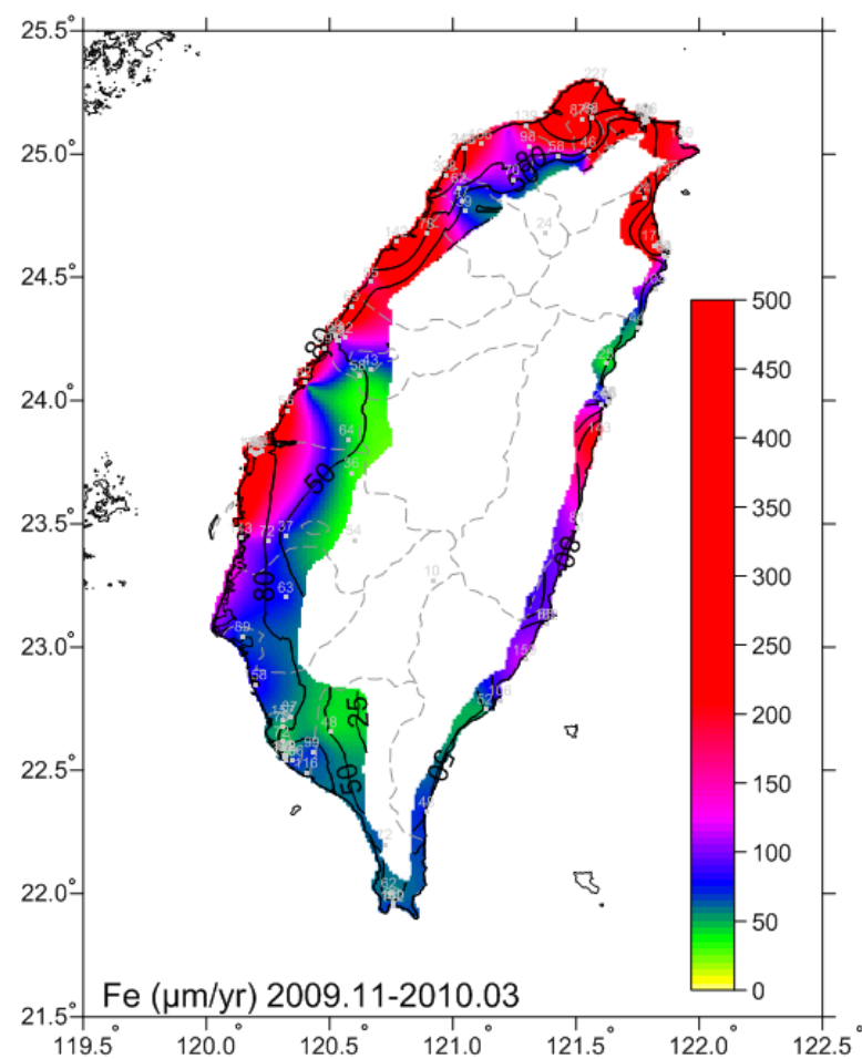
圖 6-10 2009.11-2010.03 碳鋼腐蝕速率圖
