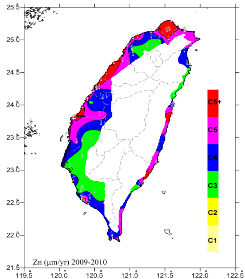
圖 6-26 2009-2010 鋅年腐蝕速率 ISO 分類圖
