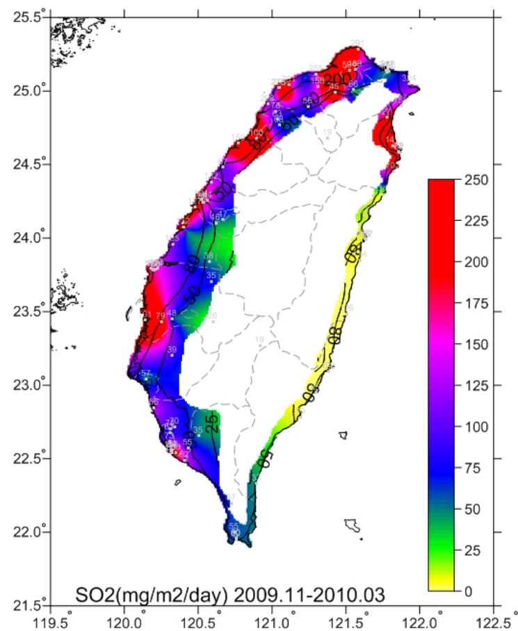
圖 5-2 2009.11-2010.03 二氧化硫沉積速率
