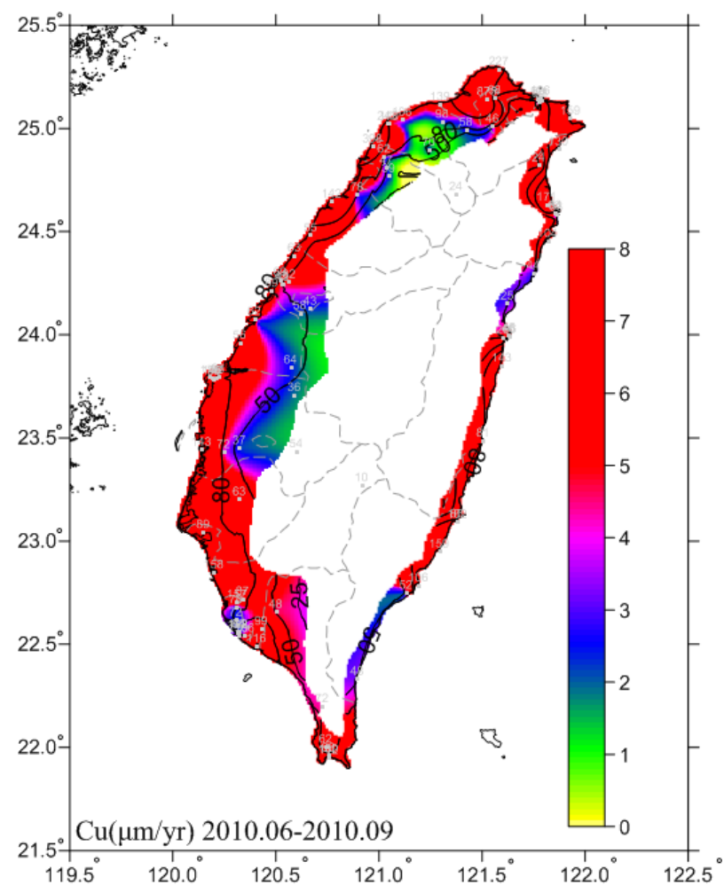
圖 6-20 2010.06-2010.09 銅腐蝕速率圖
