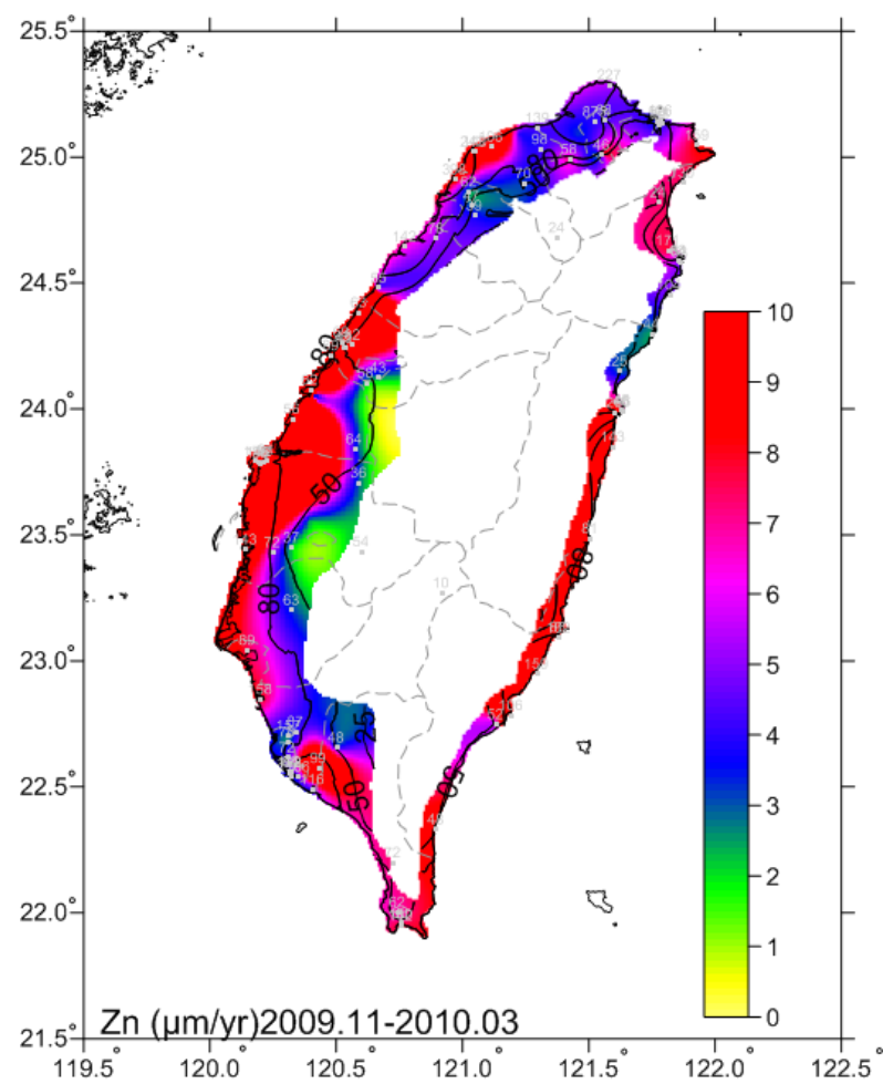
圖 6-14 2009.11-2010.03 鋅腐蝕速率圖
