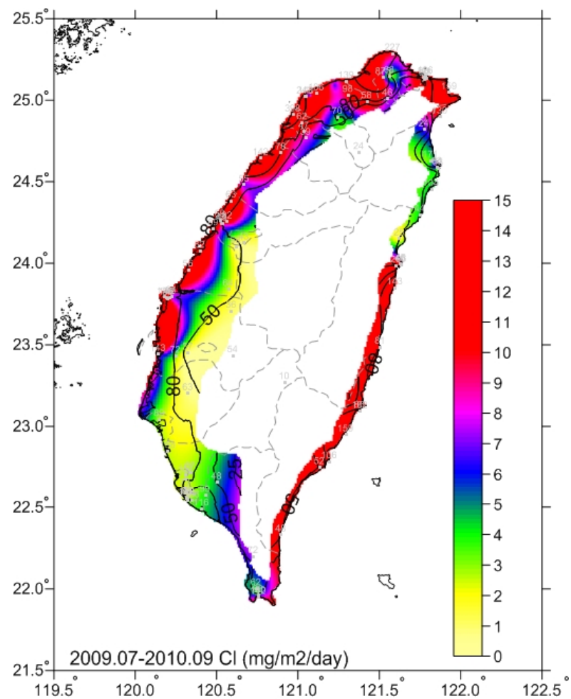
圖 4-5 2009.07-2010.09 氣鹽沉積速率圖
