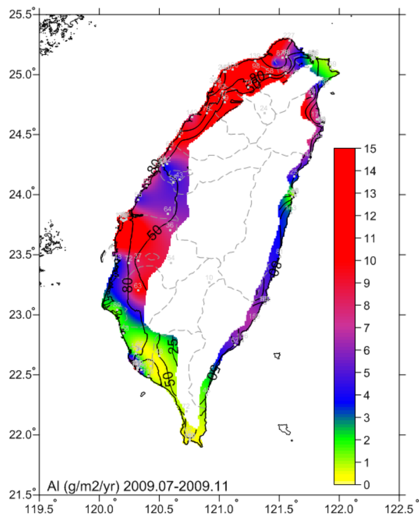
圖 6-21 2009.07-2009.11 鋁腐蝕速率圖
