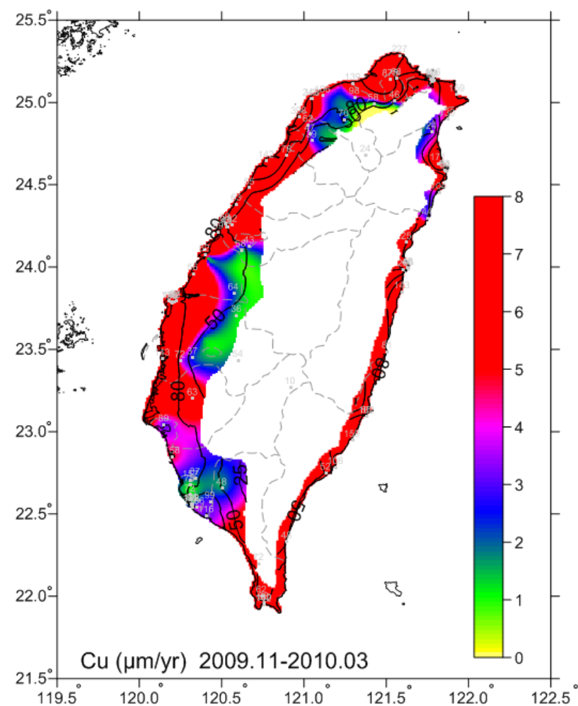
圖 6-18 2009.11-2010.03 銅腐蝕速率圖
