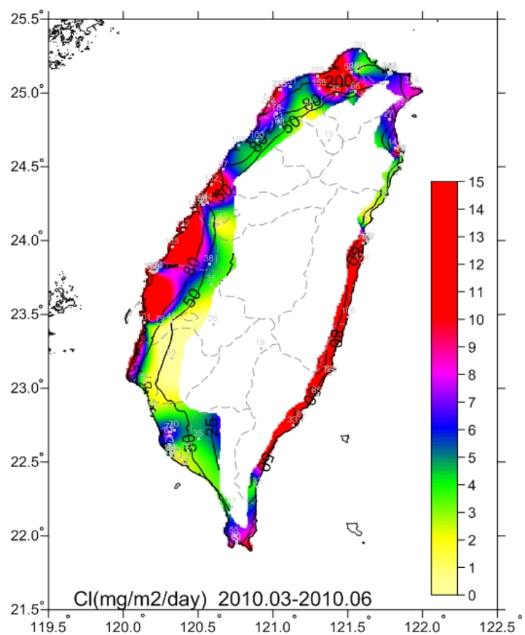
圖 4-3 2010.03-2010.06 氯鹽沉積速率圖
