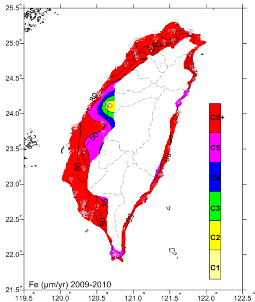
圖 6-25 2009-2010 碳鋼年腐蝕速率 ISO 分類圖
