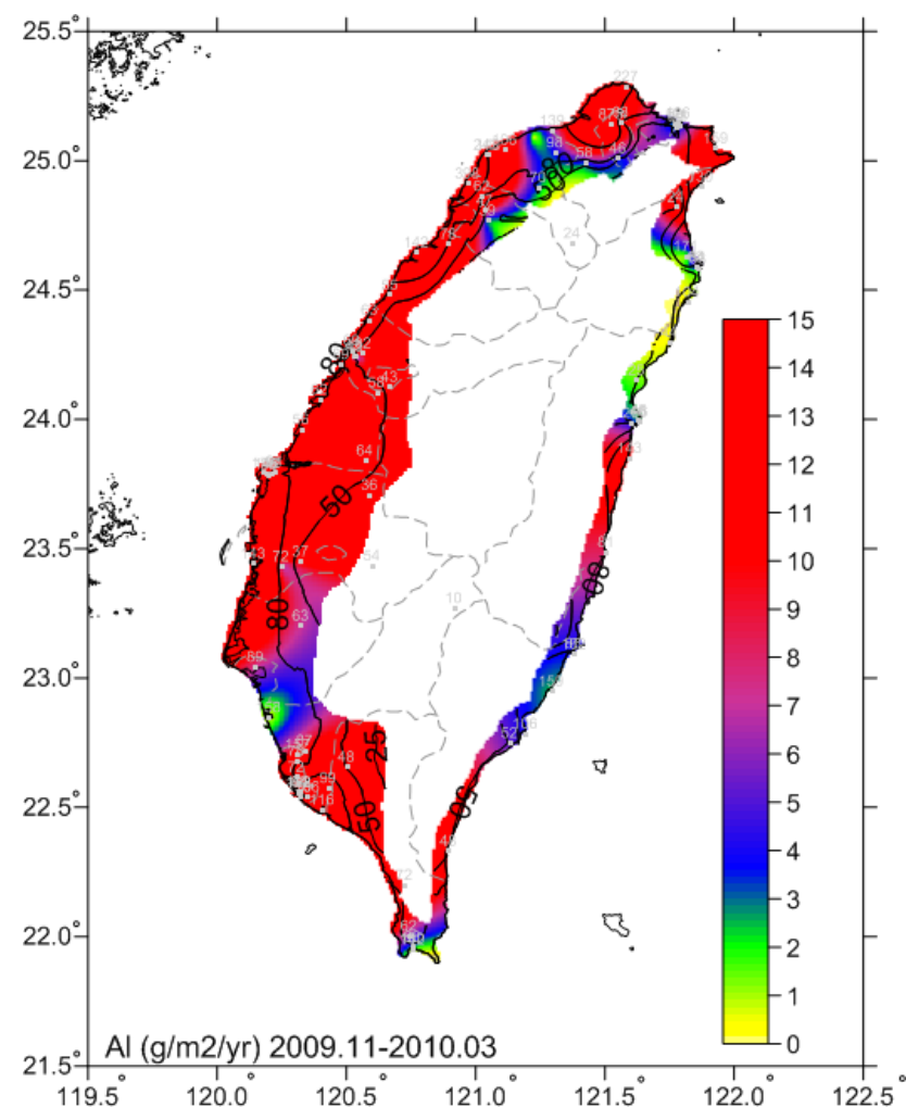
圖 6-22 2009.11-2010.03 鋁腐蝕速率圖
