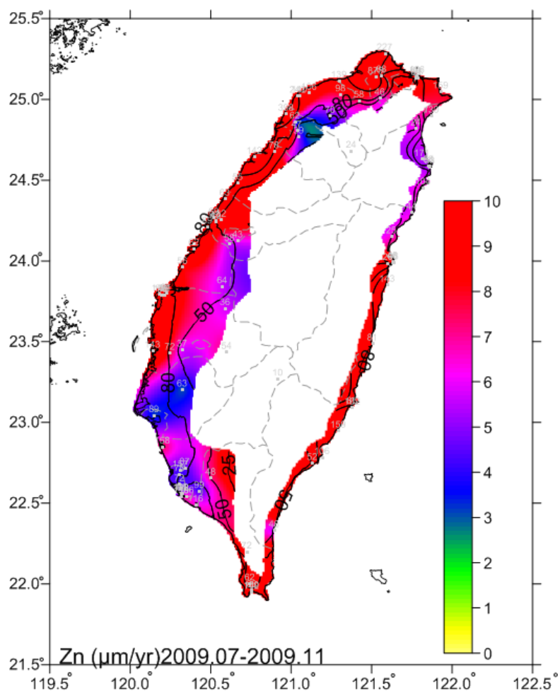
圖 6-13 2009.07-2009.11 鋅腐蝕速率圖
