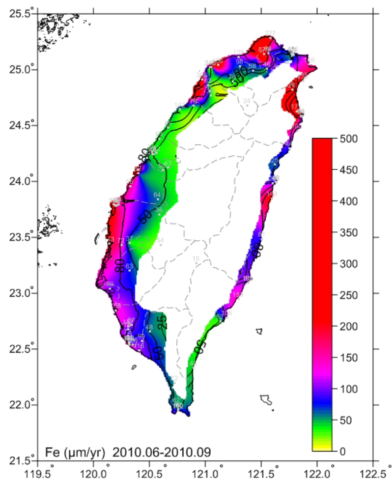
圖 6-12 2010.06-2010.09 碳鋼腐蝕速率圖
