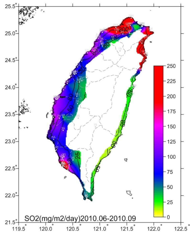
圖 5-4 2010.06-2010.09 二氧化硫沉積速率圖
