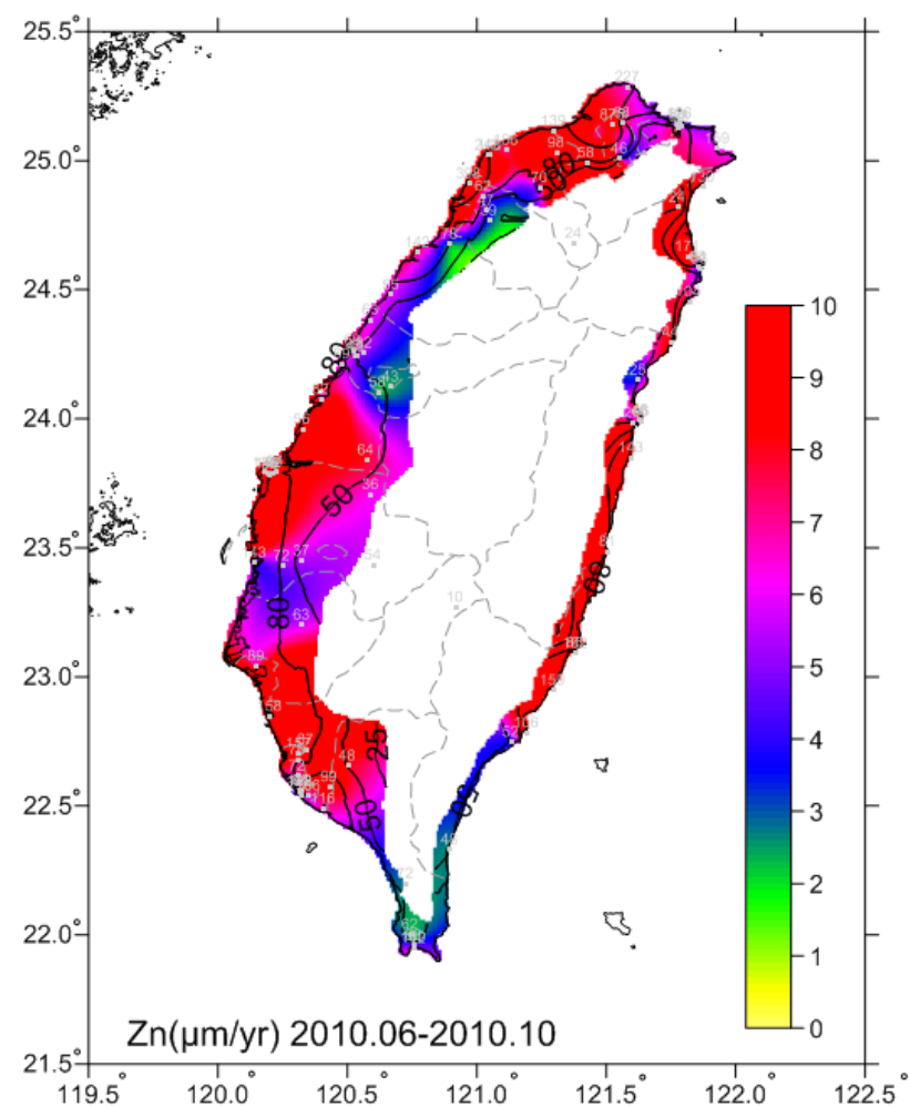
圖 6-16 2010.06-2010.10 鋅腐蝕速率圖
