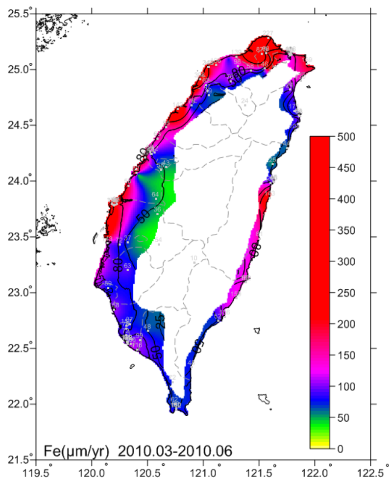
圖 6-11 2010.03-2010.06 碳鋼腐蝕速率圖
