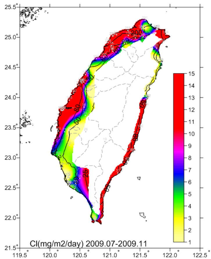
圖 4-1 2009.07-2009.11 氯鹽沉積速率圖
