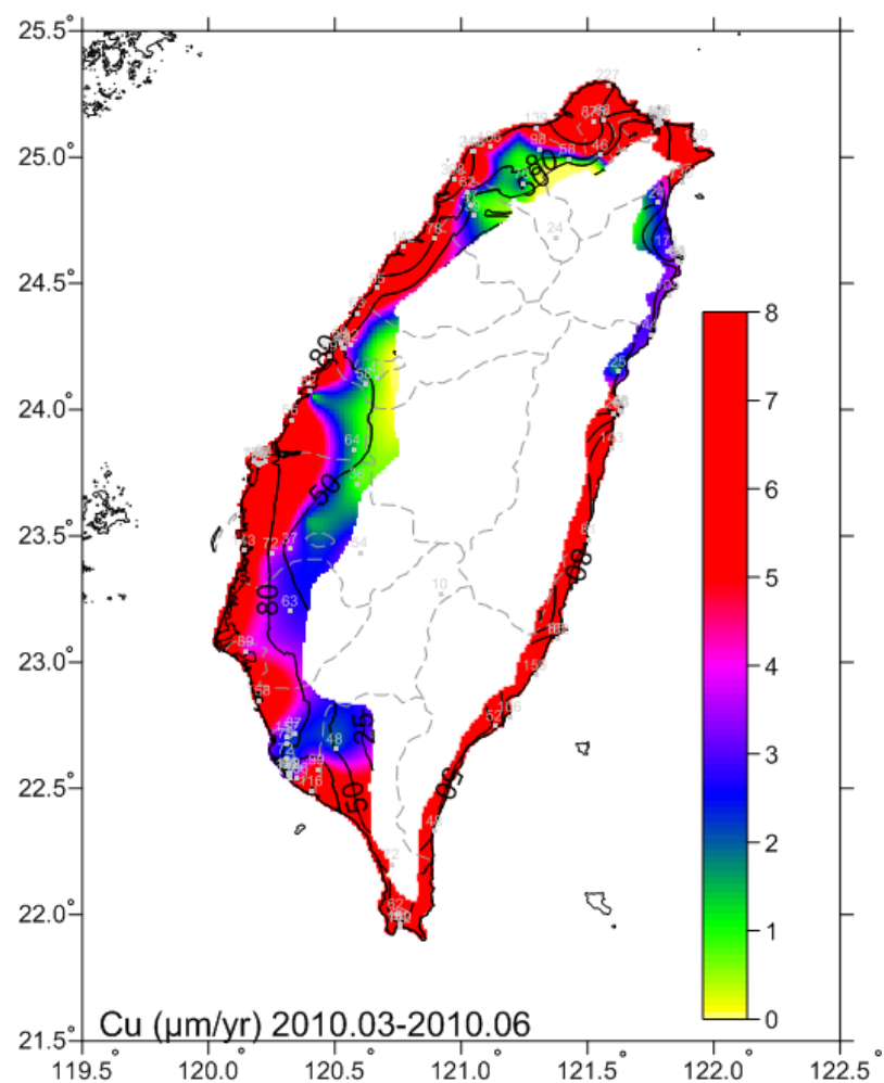
圖 6-19 2010.03-2010.06 銅腐蝕速率圖
