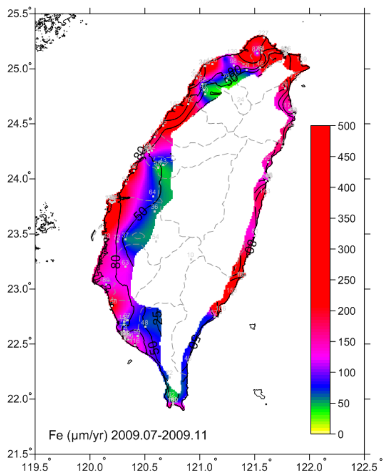
圖 6-9 2009.07-2009.11 碳鋼腐蝕速率圖
