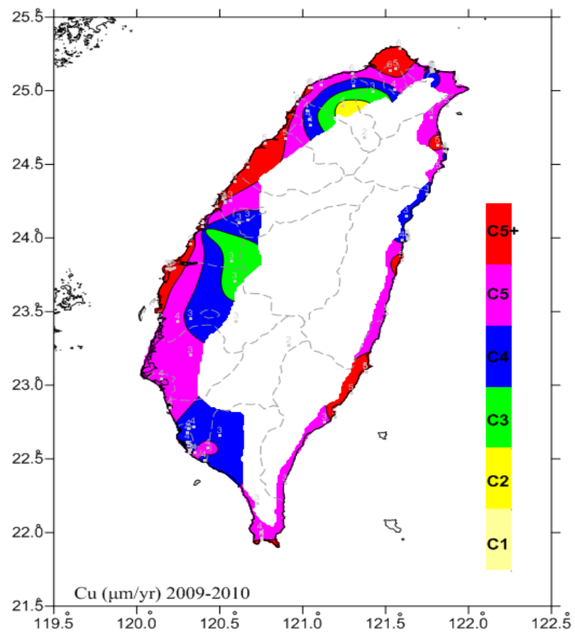
圖 6-27 2009-2010 銅年腐蝕速率 ISO 分類圖
