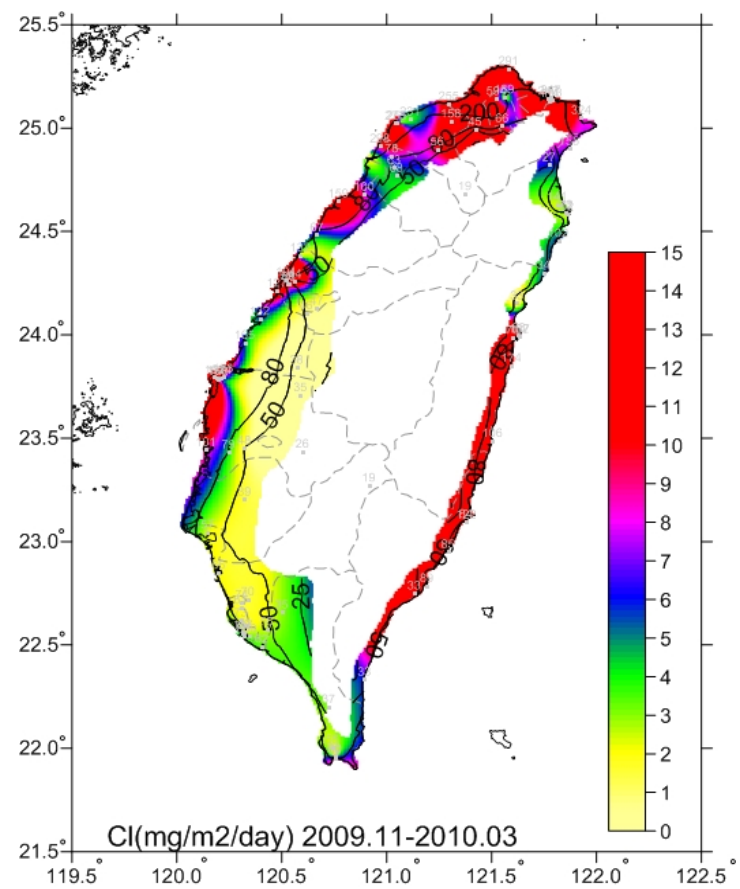
圖 4-2 2009.11-2010.03 氯鹽沉積速率圖
