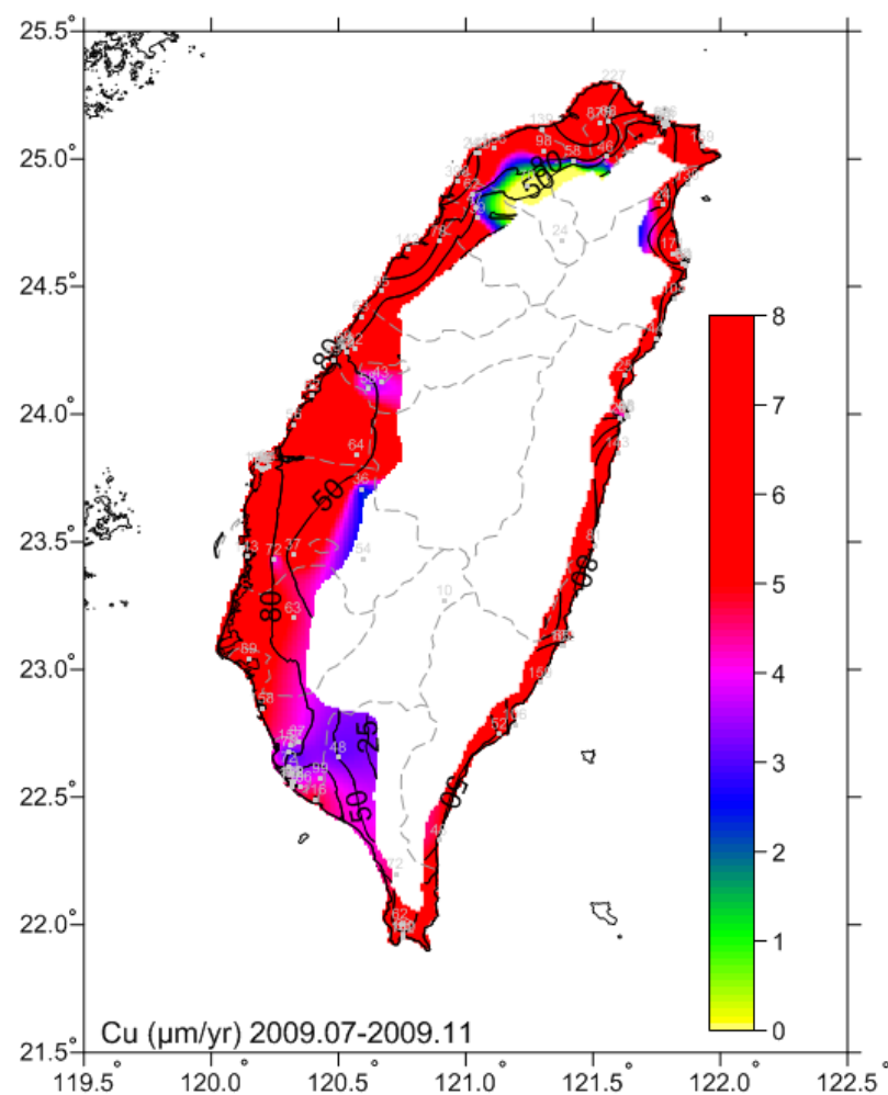
圖 6-17 2009.07-2009.11 銅腐蝕速率圖
