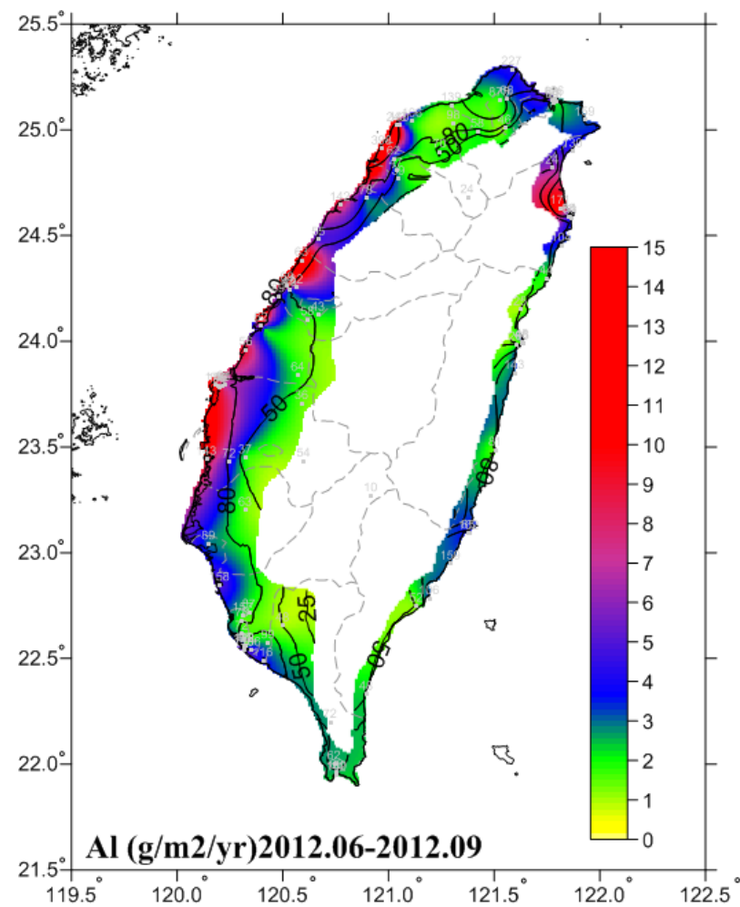
圖 6-24 2012.06-2012.09 鋁腐蝕速率圖
