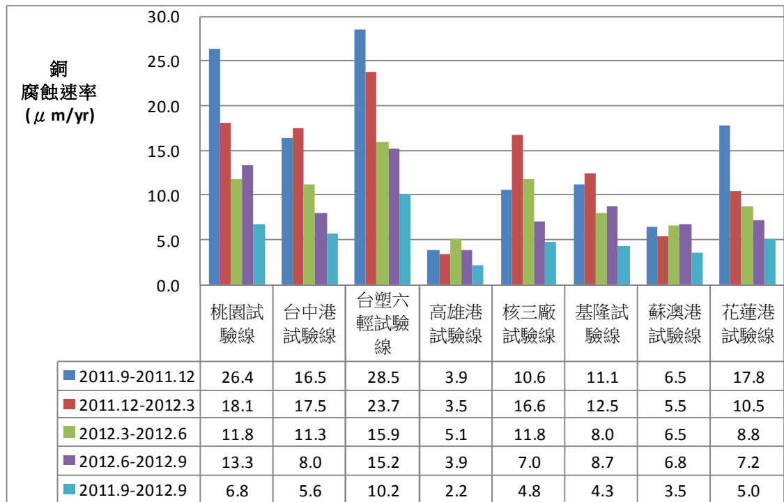
圖 6-3 垂直海岸試驗線銅腐蝕速率比較圖
