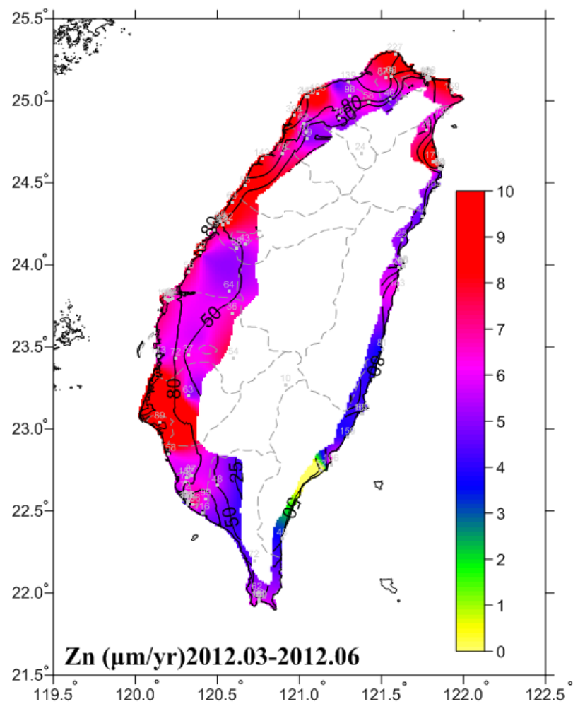
圖 6-15 2012.03-2012.06 鋅腐蝕速率圖
