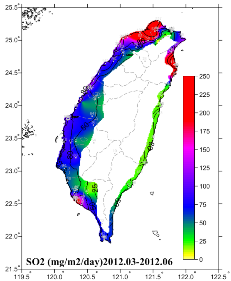
圖 5-3 2012.03-2012.06 二氧化硫沉積速率圖
