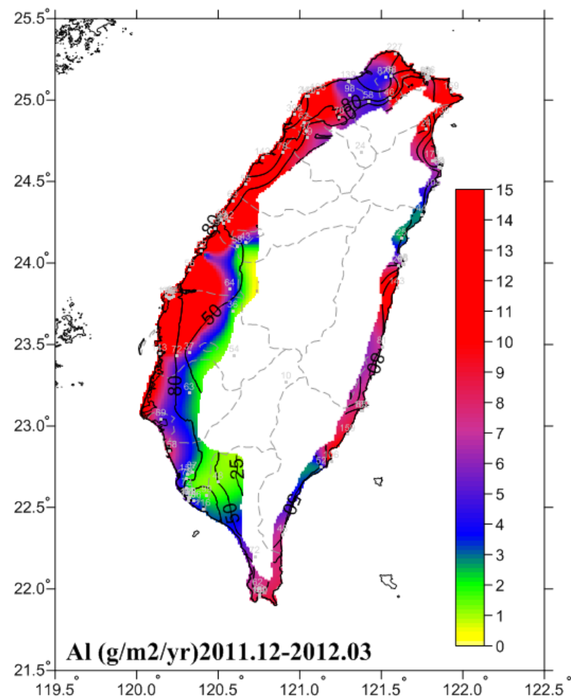
圖 6-22 2011.12-2012.03 鋁腐蝕速率圖
