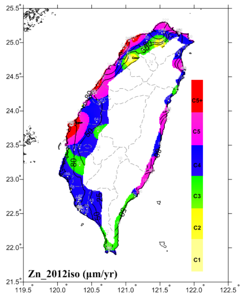
圖 6-26 2012 鋅年腐蝕速率 ISO 分類圖
