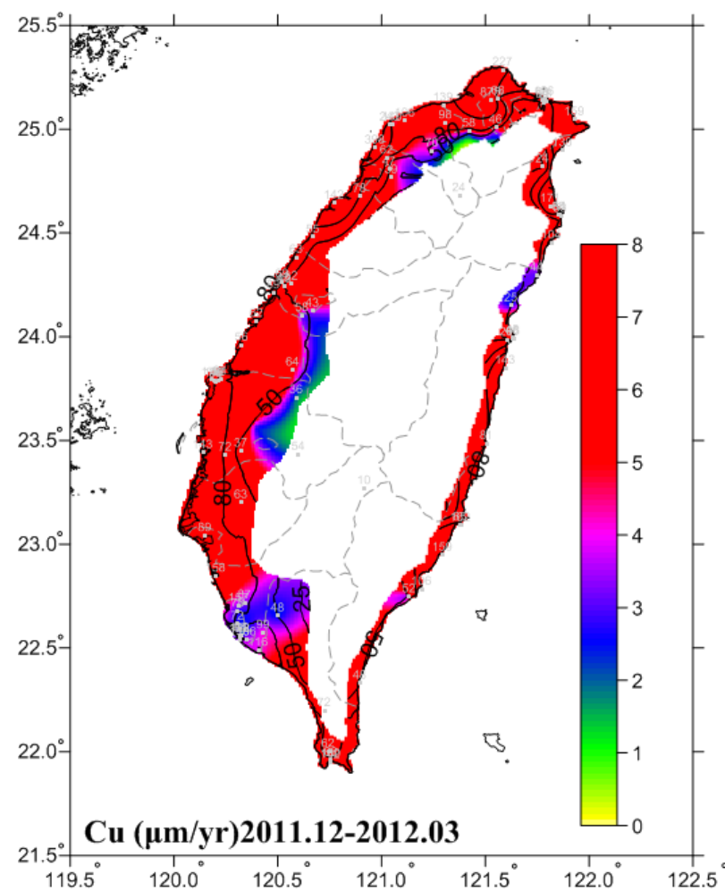
圖 6-18 2011.12-2012.03 銅腐蝕速率圖
