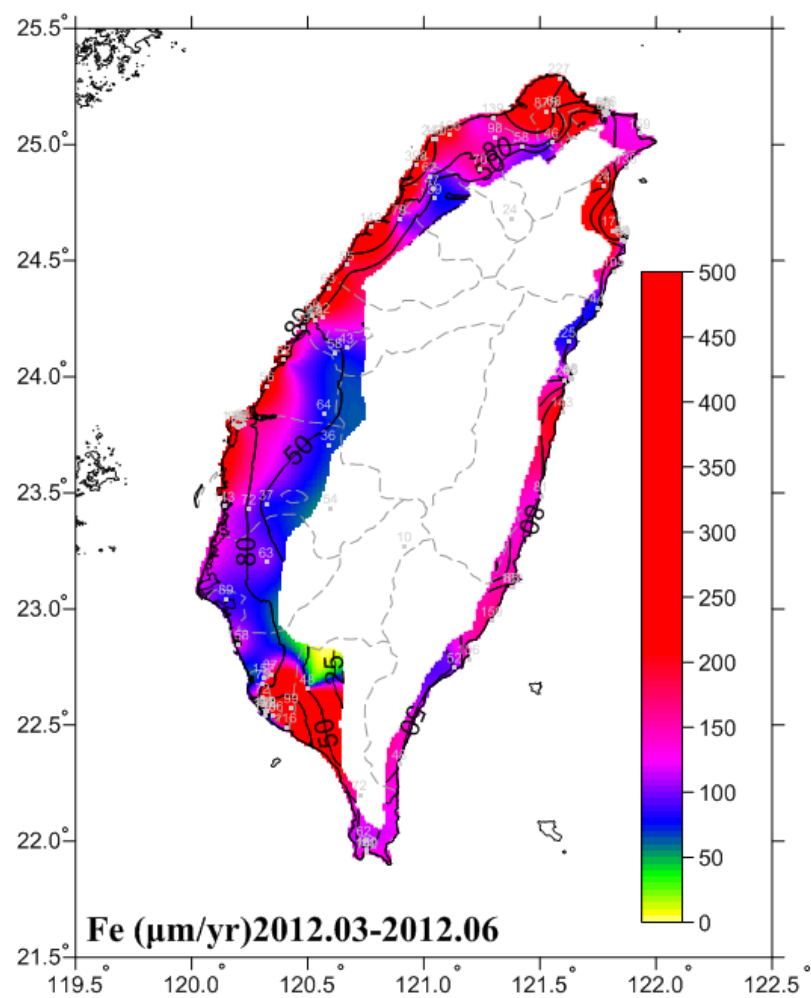
圖 6-11 2012.03-2012.06 碳鋼腐蝕速率圖
