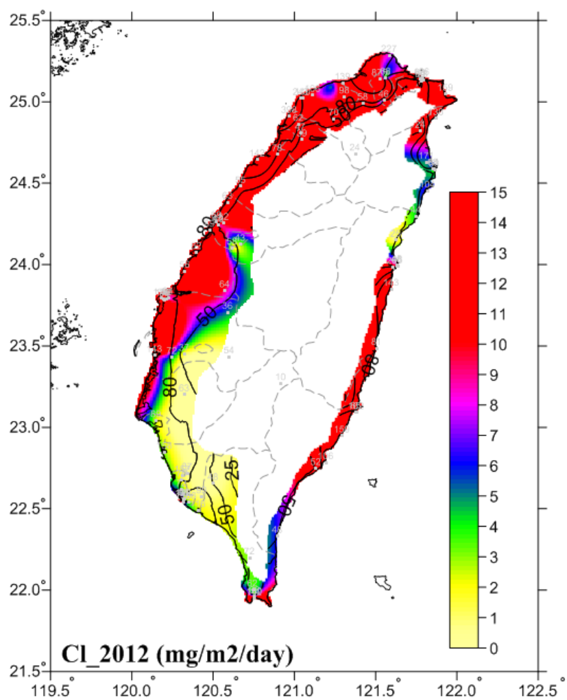
圖 4-5 2012 氣鹽沉積速率圖
