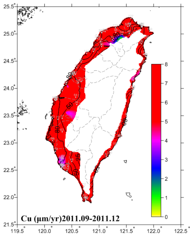
圖 6-17 2011.09-2011.12 銅腐蝕速率圖
