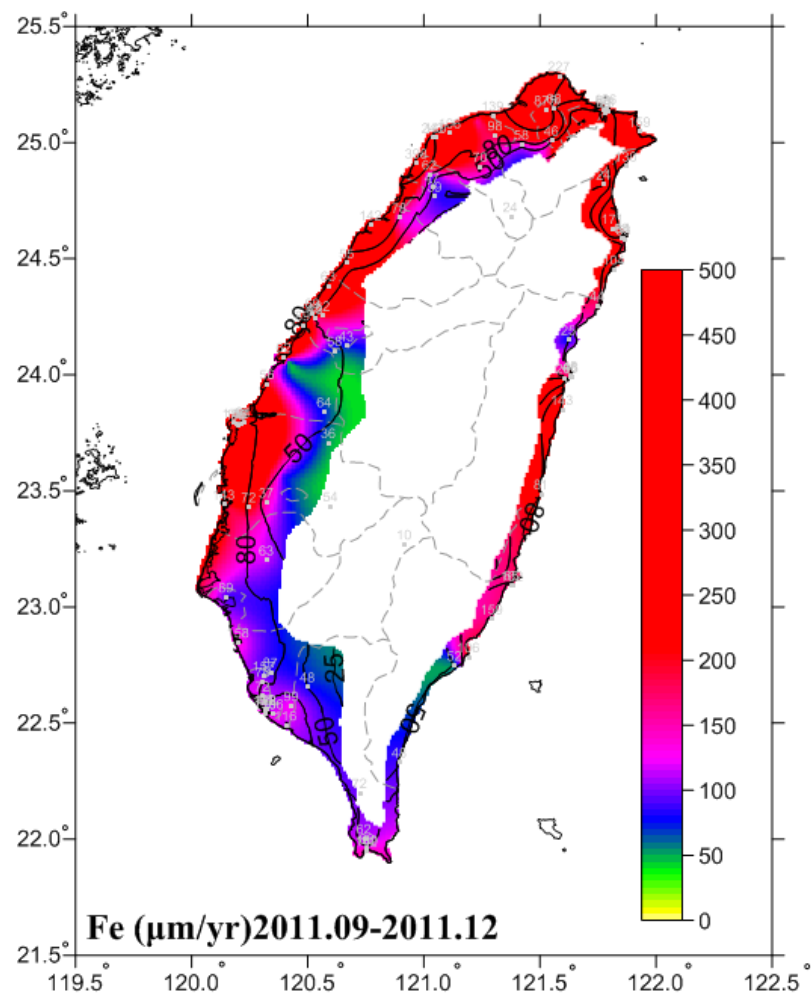
圖 6-9 2011.09-2011.12 碳鋼腐蝕速率圖
