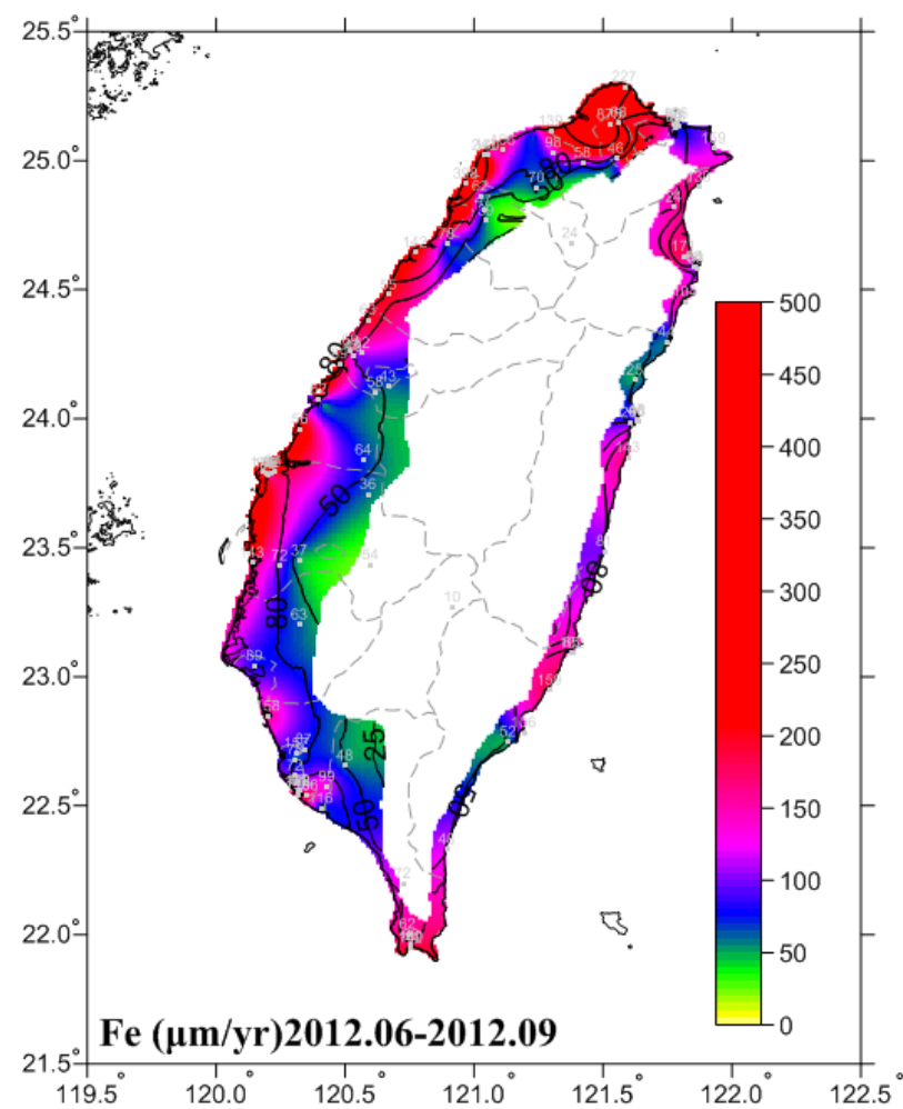
圖 6-12 2012.06-2012.09 碳鋼腐蝕速率圖
