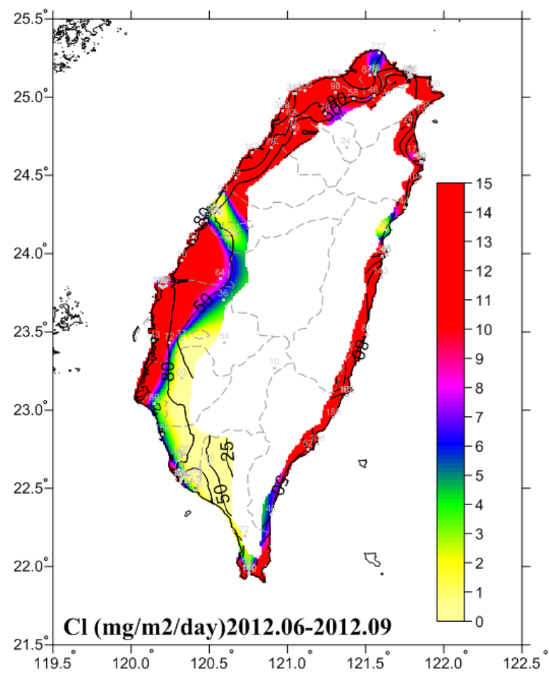
圖 4-4 2012.06-2012.09 氯鹽沉積速率圖
