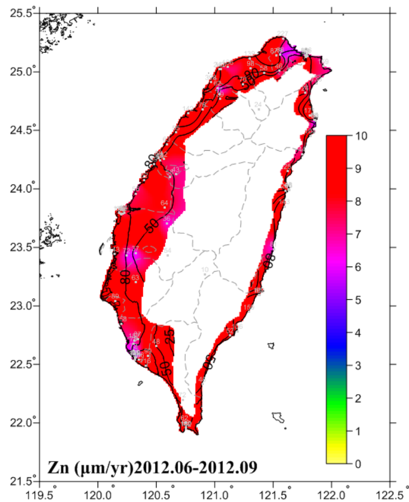
圖 6-16 2012.06-2012.09 鋅腐蝕速率圖
