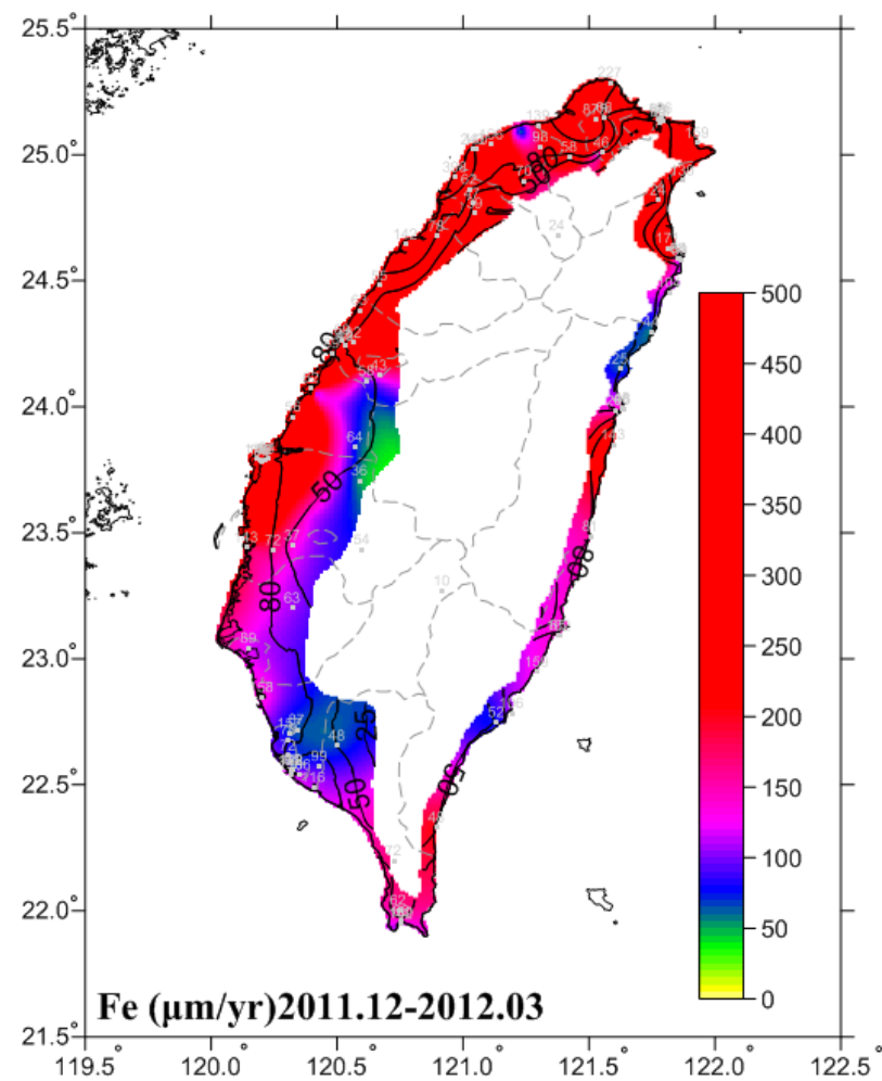
圖 6-10 2011.12-2012.03 碳鋼腐蝕速率圖
