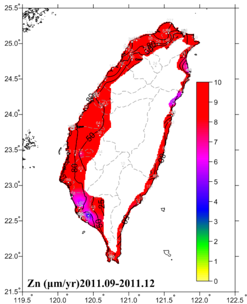
圖 6-13 2011.09-2011.12 鋅腐蝕速率圖
