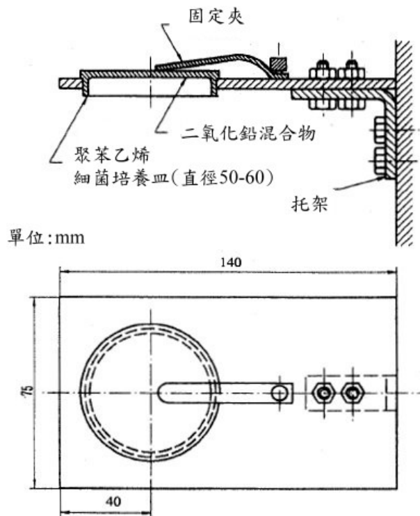
圖 1-3 二氧化硫沉積量採集裝置
