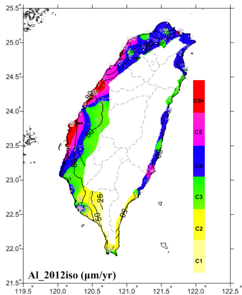
圖 6-28 2012 鋁年腐蝕速率 ISO 分類圖
