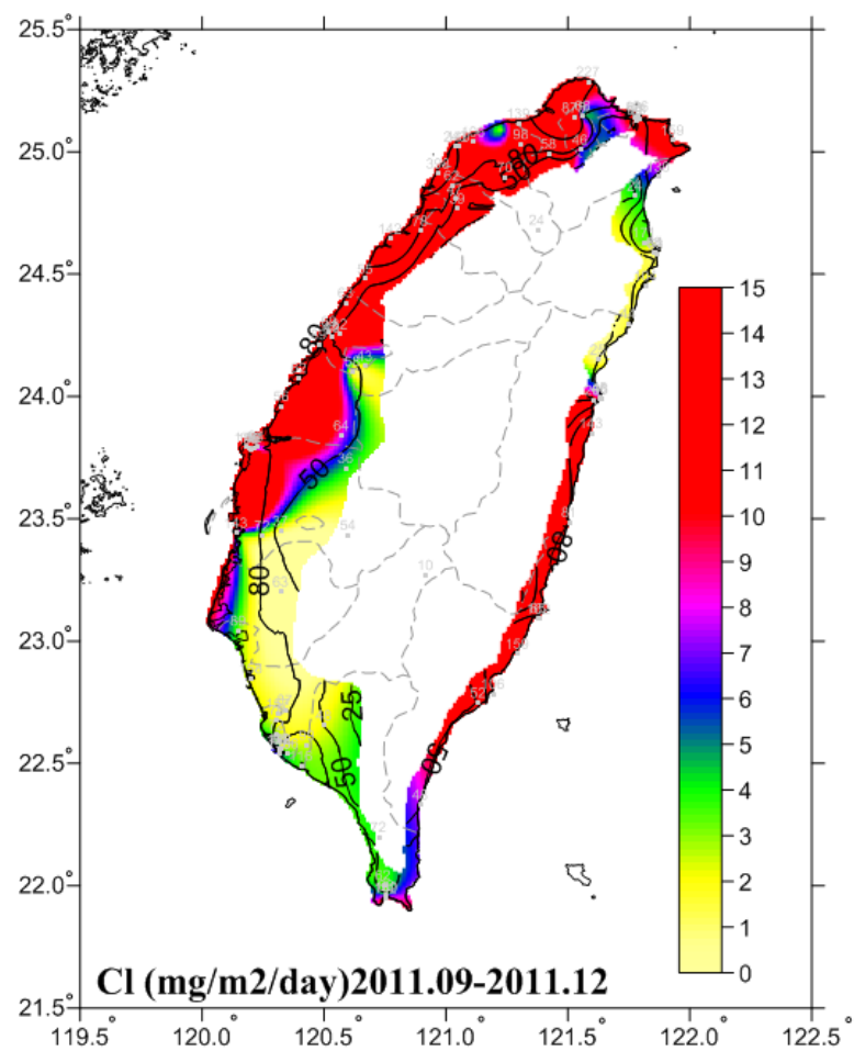
圖 4-1 2011.09-2011.12 氯鹽沉積速率圖
