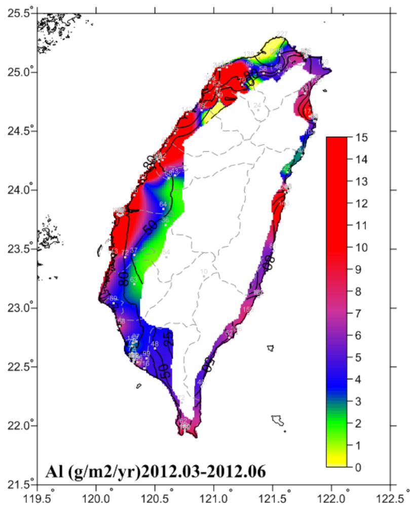
圖 6-23 2012.03-2012.06 鋁腐蝕速率圖
