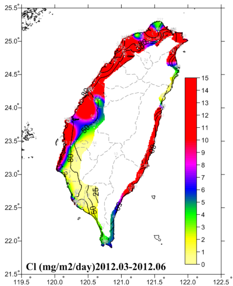
圖 4-3 2012.03-2012.06 氯鹽沉積速率圖
