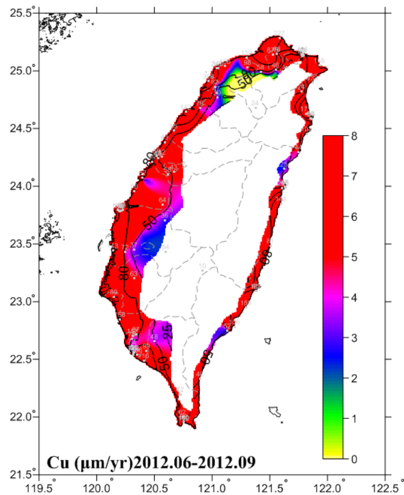
圖 6-20 2012.06-2012.09 銅腐蝕速率圖
