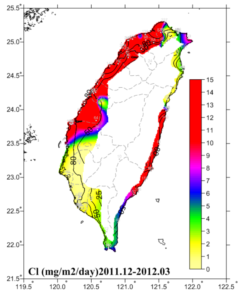
圖 4-2 2011.12-2012.03 氯鹽沉積速率圖
