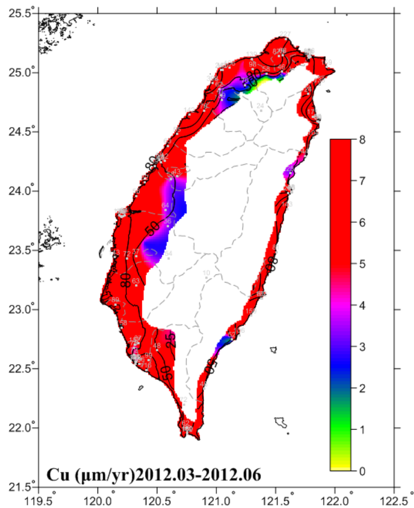
圖 6-19 2012.03-2012.06 銅腐蝕速率圖
