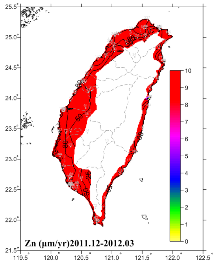
圖 6-14 2011.12-2012.03 鋅腐蝕速率圖
