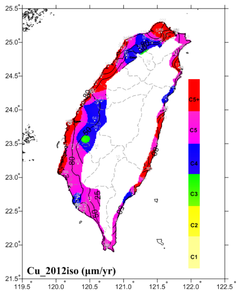
圖 6-27 2012 銅年腐蝕速率 ISO 分類圖
