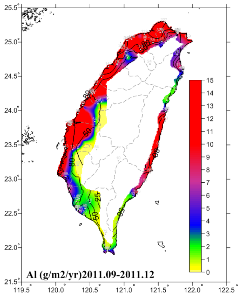
圖 6-21 2011.09-2011.12 鋁腐蝕速率圖
