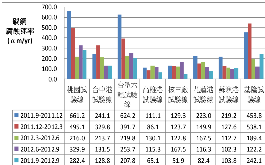
圖 6-1 垂直海岸試驗線碳鋼腐蝕速率比較圖
