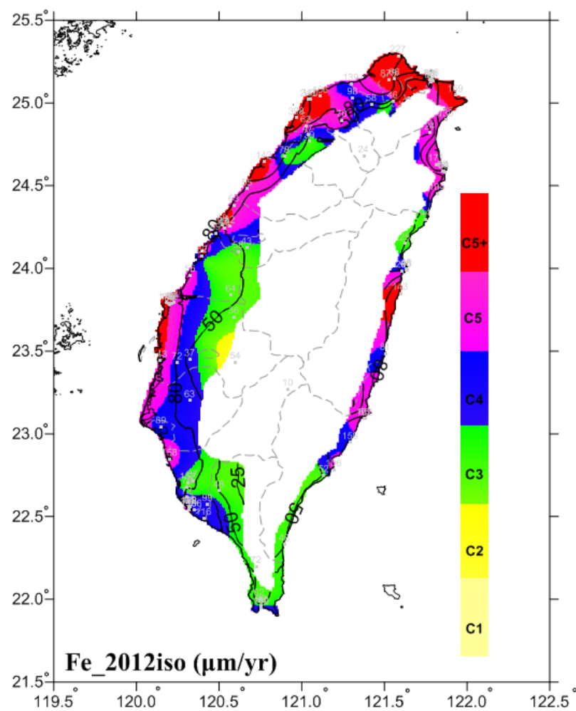
圖 6-25 2012 碳鋼年腐蝕速率 ISO 分類圖
