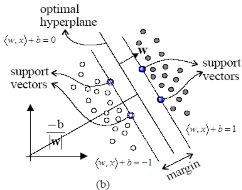
圖 2.4 最大分離間隔與最優分離超平面 (Yonas B. Dibike1.等，2000)
