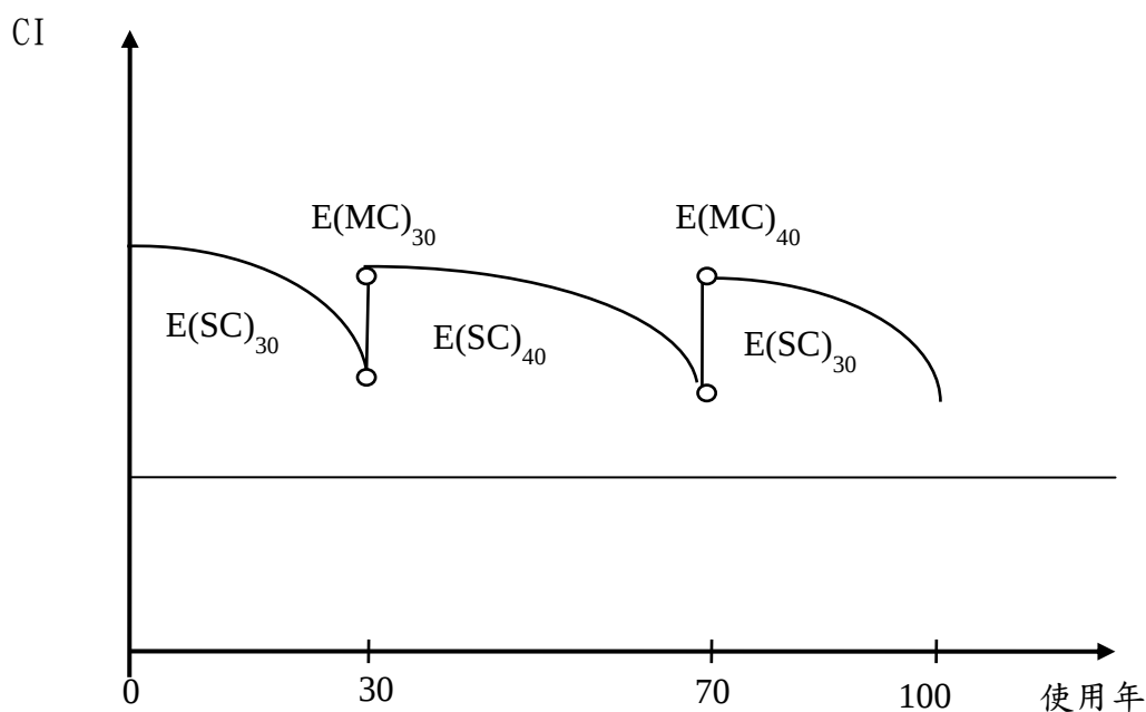
圖6.5 橋梁在第30年與第70年維護策略
