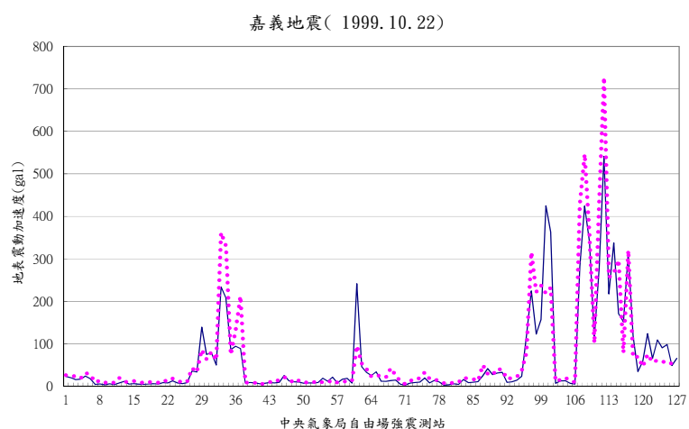
圖 4.14 臺灣歷年大地震:嘉義地震之實測值與預測值比較
