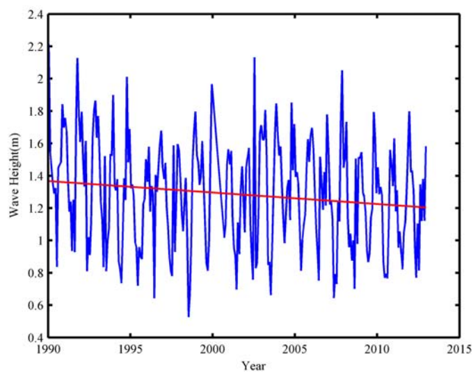
圖 2.6 花蓮港月平均波浪資料及其趨勢線
