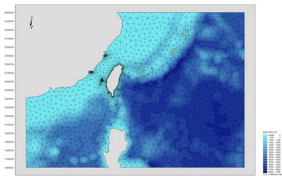
二維數值模式計算網格範圍
