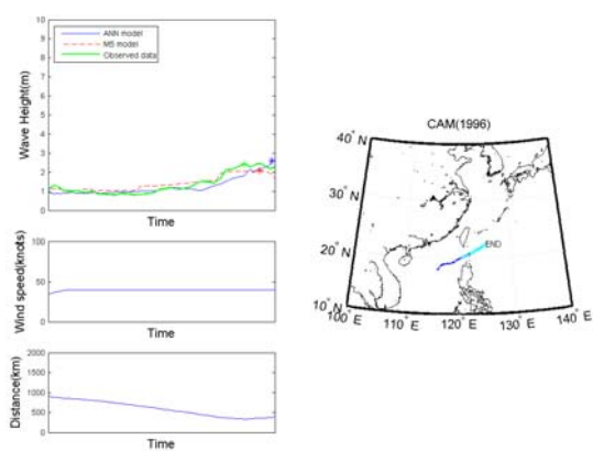
附圖 16 凱姆(1996)颱風資訊與花蓮港推算結果
