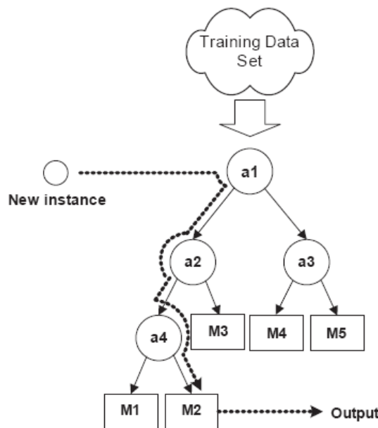
圖 4.1 層級模組法示意圖(ai 為屬性，Mi 為分群之模組)
