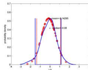
二維數值模式模擬花蓮港颱風波浪驗證結果
