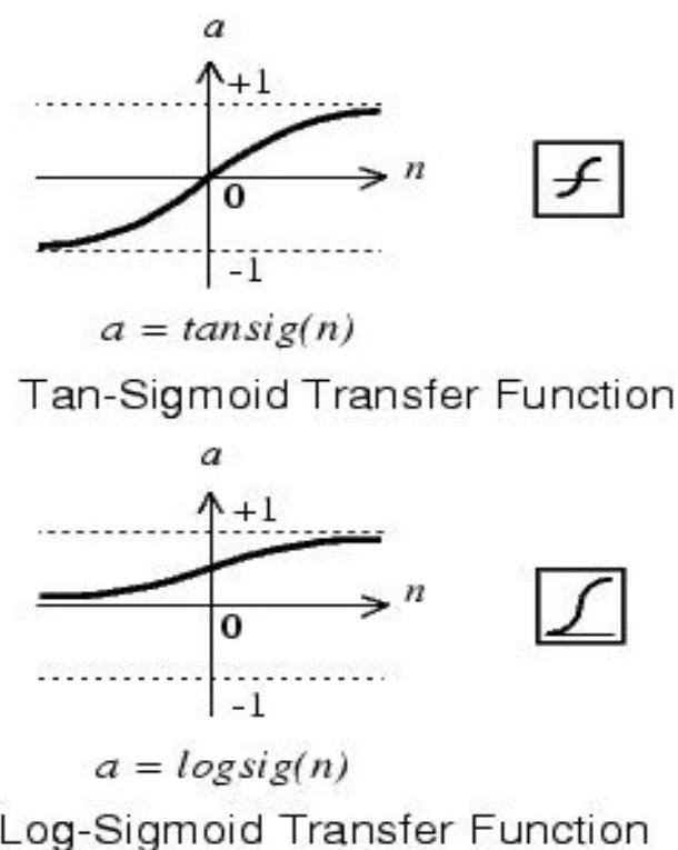
圖 3.7 正切雙彎曲轉換函數與雙彎曲函數
