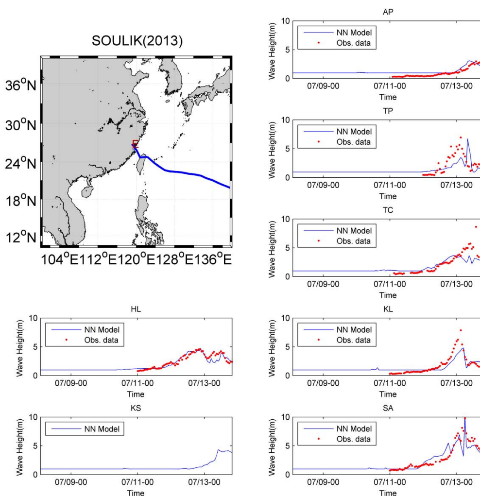
附圖 122 蘇力颱風各主要港口颱風波浪推算結果
