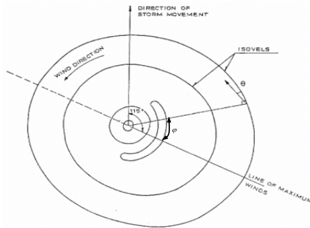
圖 3.4 氣旋中心附近風速風向分佈示意圖
