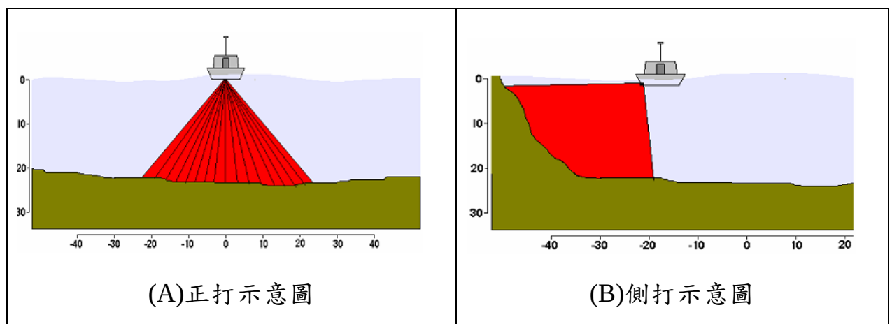
圖 3.13 多音束水深測量音鼓正打側打差異示意圖
