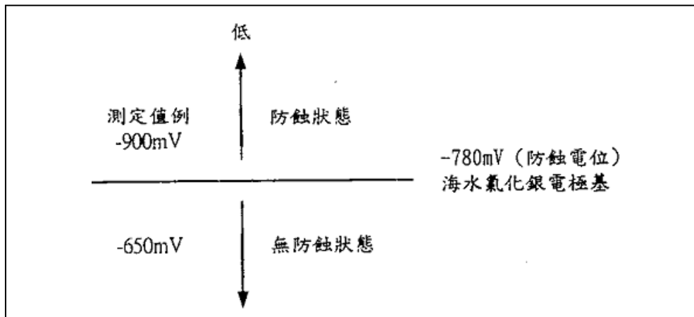
圖 3.19 防蝕效果的判定方法
