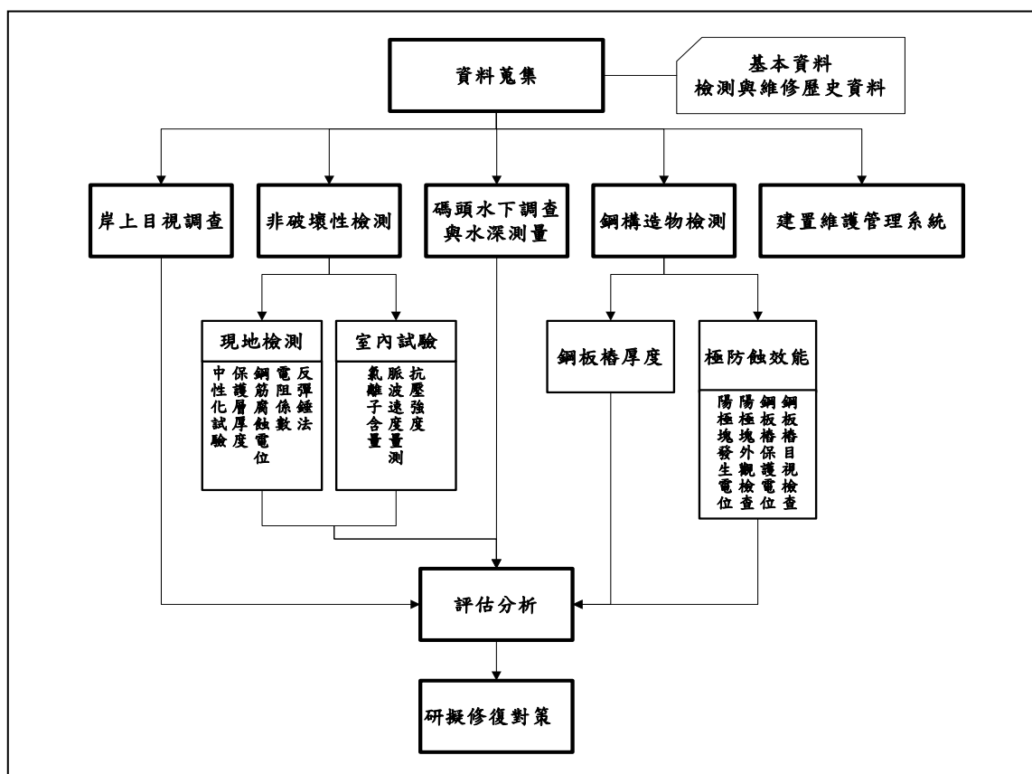
圖 3.1 現況調查流程
