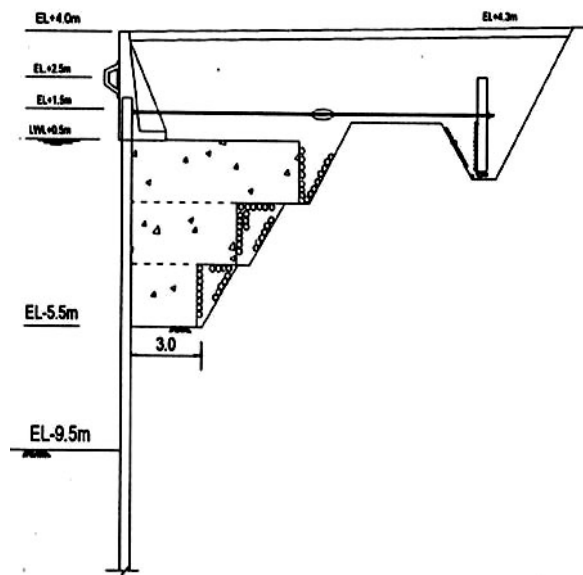
花蓮港 9 號碼頭結構型式
