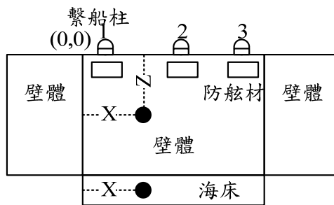
圖 2.4 重力或板樁式碼頭正視圖
