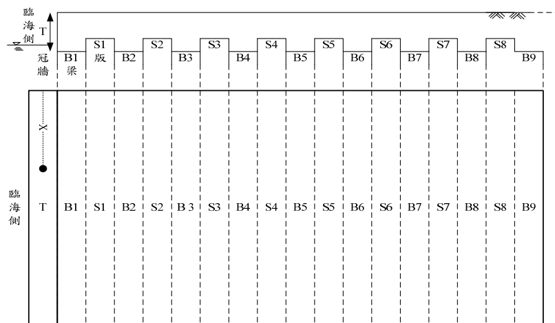
圖 2.6 棧橋式碼頭岸肩底部梁版編號示意
