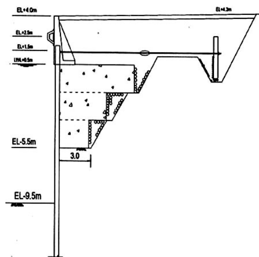
圖 4.33 9 號碼頭結構斷面圖
