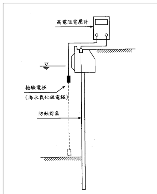
圖 3.20 電位測定示意圖
