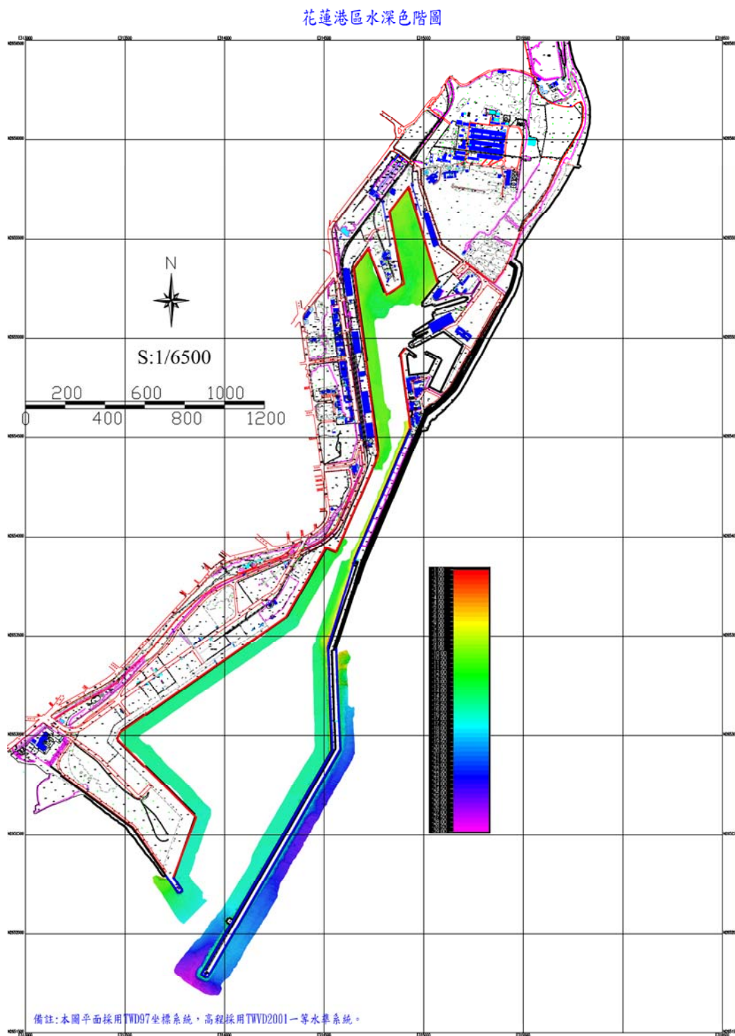
圖 4.19 花蓮港港區水深測量色階圖
