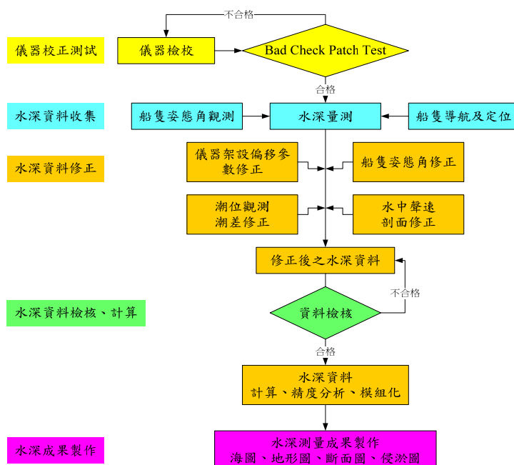
圖 3.17 水深測量作業流程圖
