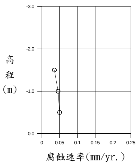
圖 4.30 7 號登陸碼頭鋼板樁腐蝕速率與水深之關係
