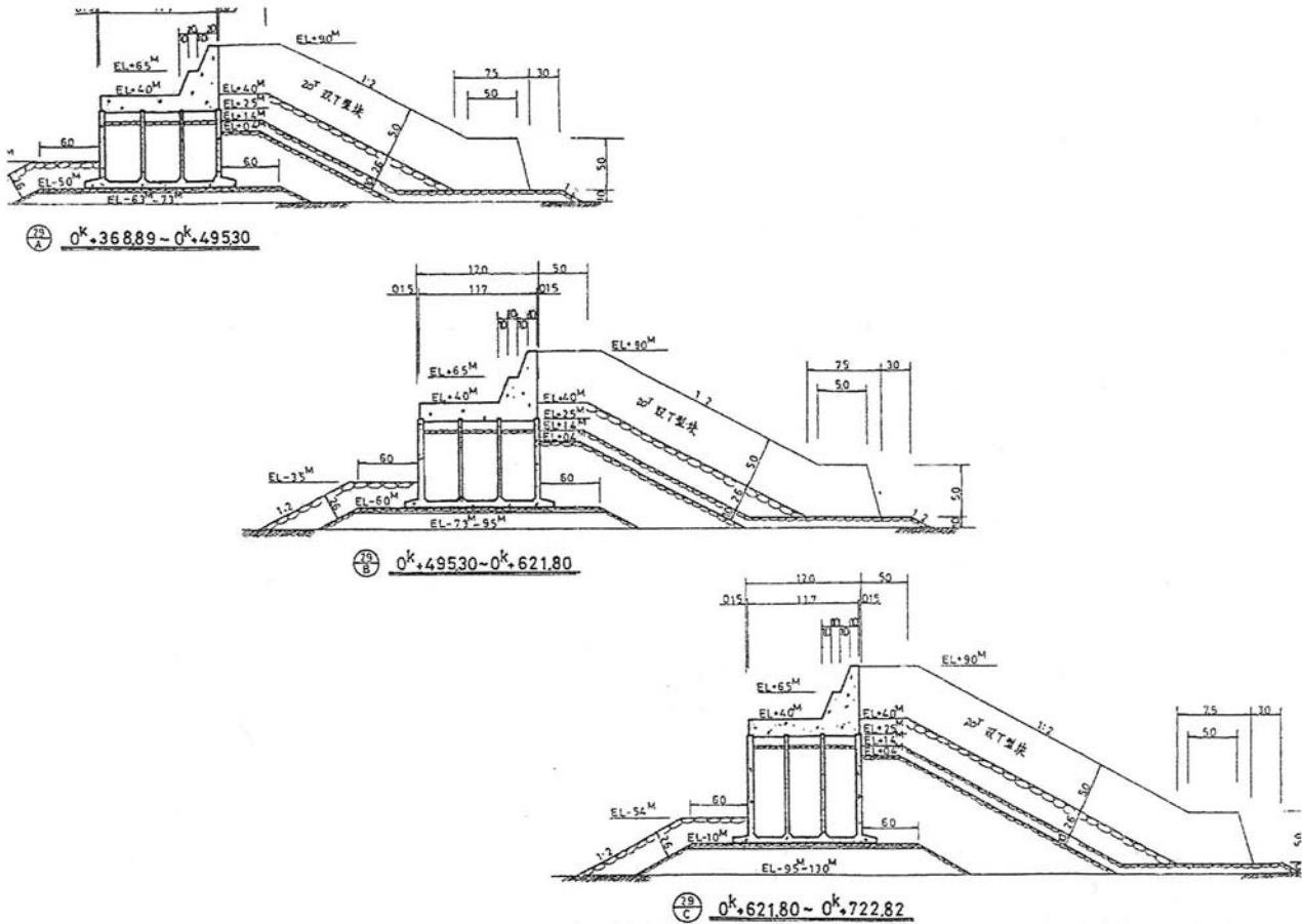
西防波堤結構型式
