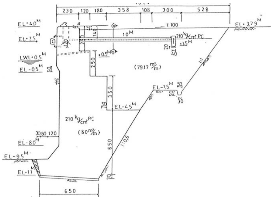
花蓮港 10、11、13、14 號碼頭結構型式
