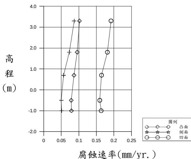
圖 4.26 5 號碼頭鋼板樁腐蝕速率與水深之關係
