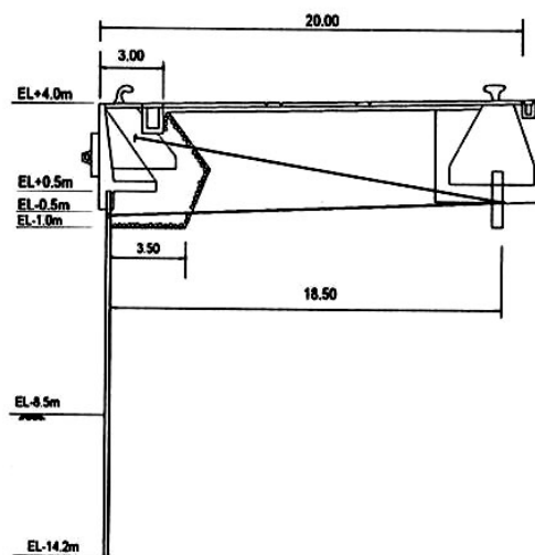
圖 4.27 6 號碼頭結構斷面圖
