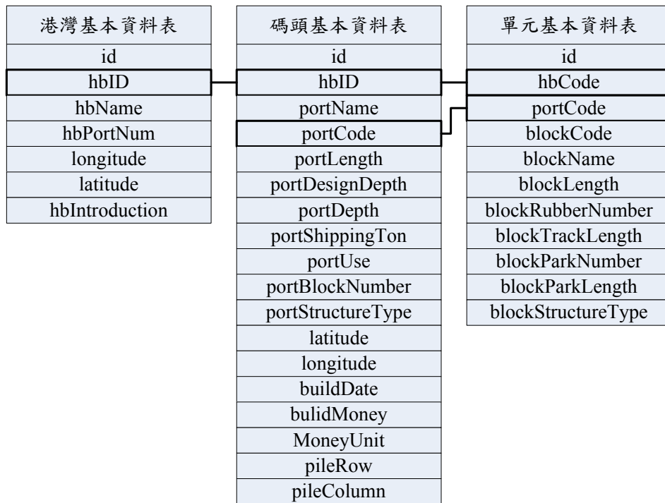
圖 4.39 關聯式查詢方式示意
