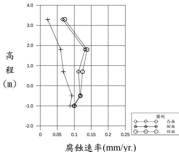
圖 4.22 4 號碼頭鋼板樁腐蝕速率與水深(高程)之關係
