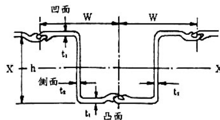
圖 4.21 Z 型鋼板樁型式圖
