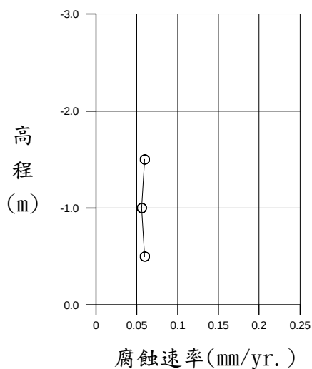
圖 4.35 9 號碼頭鋼板樁腐蝕速率與水深之關係
