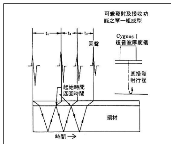
圖 3.18 測厚儀量測之示意圖
