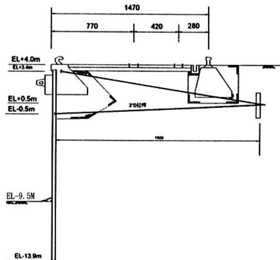
圖 4.20 4 號、5 號碼頭結構斷面圖
