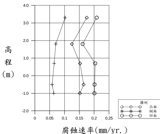
圖 4.28 6 號碼頭鋼板樁腐蝕速率與水深之關係
