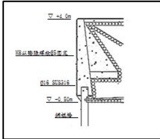
圖 4.25 電位量測導桿位置安裝示意圖
