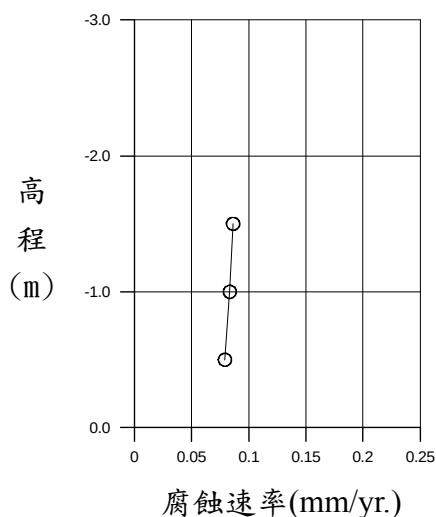
圖 4.32 8 號碼頭鋼板樁腐蝕速率與水深之關係
