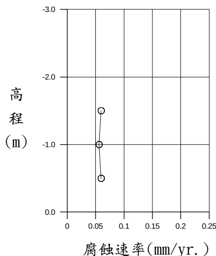
圖 4.37 航道西側岸壁鋼板樁腐蝕速率與水深之關係
