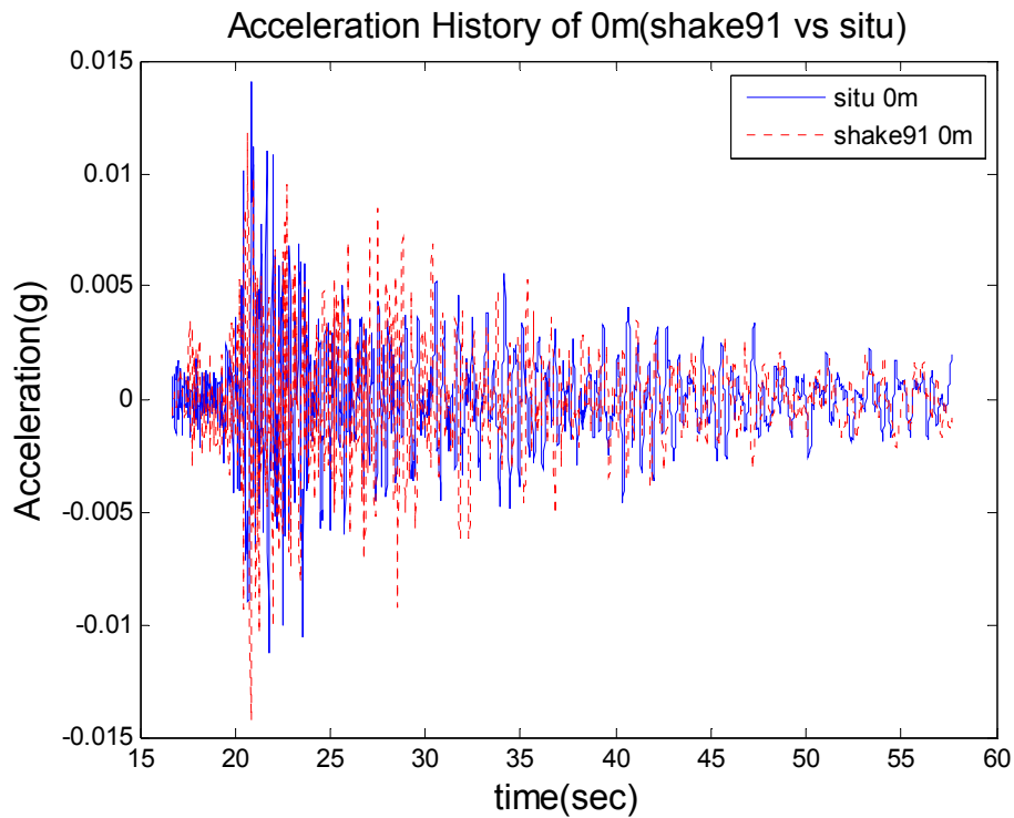
圖 3.34a 現地與 Shake91 加速度歷時比較圖(地表)
