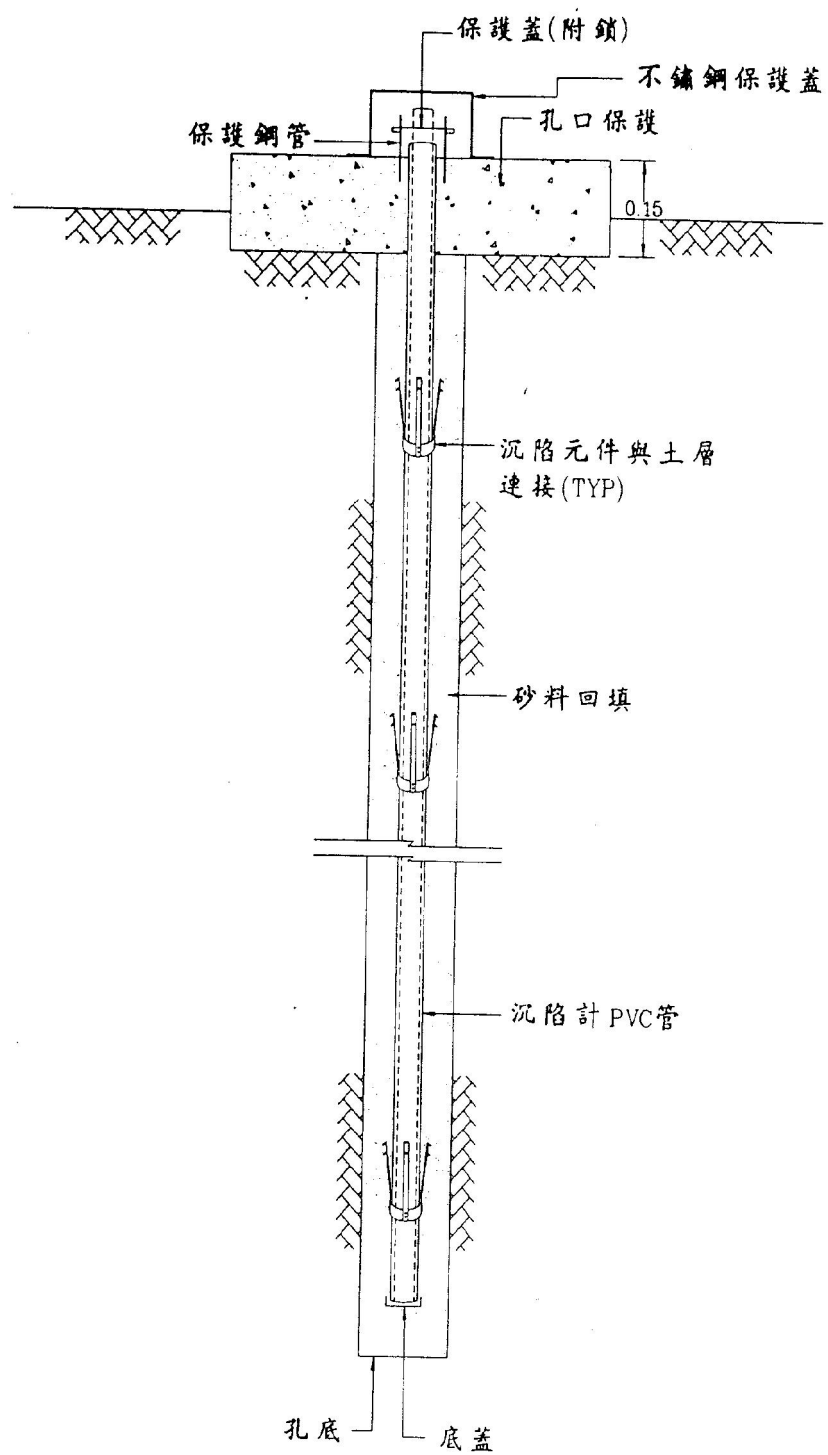
圖 2.19 磁感式層別沉陷計安裝示意圖
