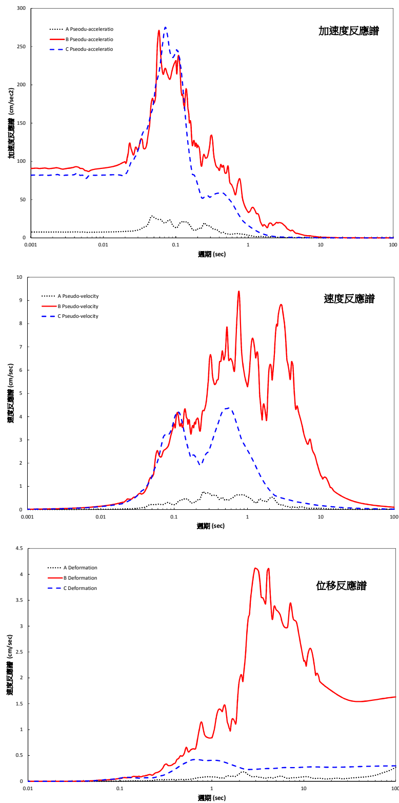
圖 3.14 安平港 A、B 及 C 類型地震之加速度、速度及位移反應譜圖
