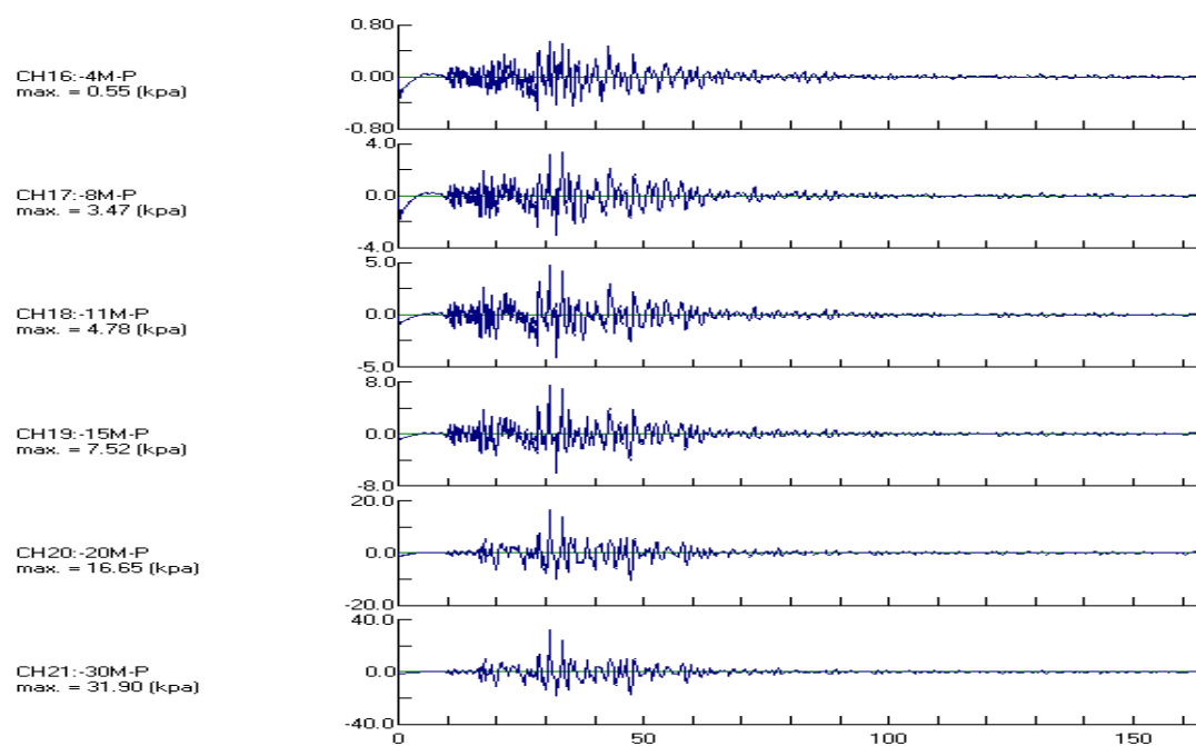
圖 3.54b 安平港 2010 年 3 月 4 日地震之動態孔隙水壓變化 (大於 0.08Hz)
