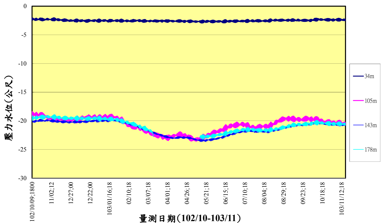
5.7c 布袋港分層水位變化圖(自記式)
