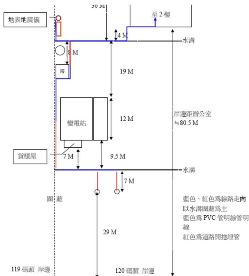
圖 4.1 高雄港 120 號碼頭動態監測站配置
