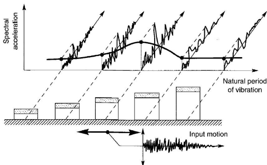
圖 3.32 單自由度系統之加速度反應示意圖(Kramer,1996) [9]
