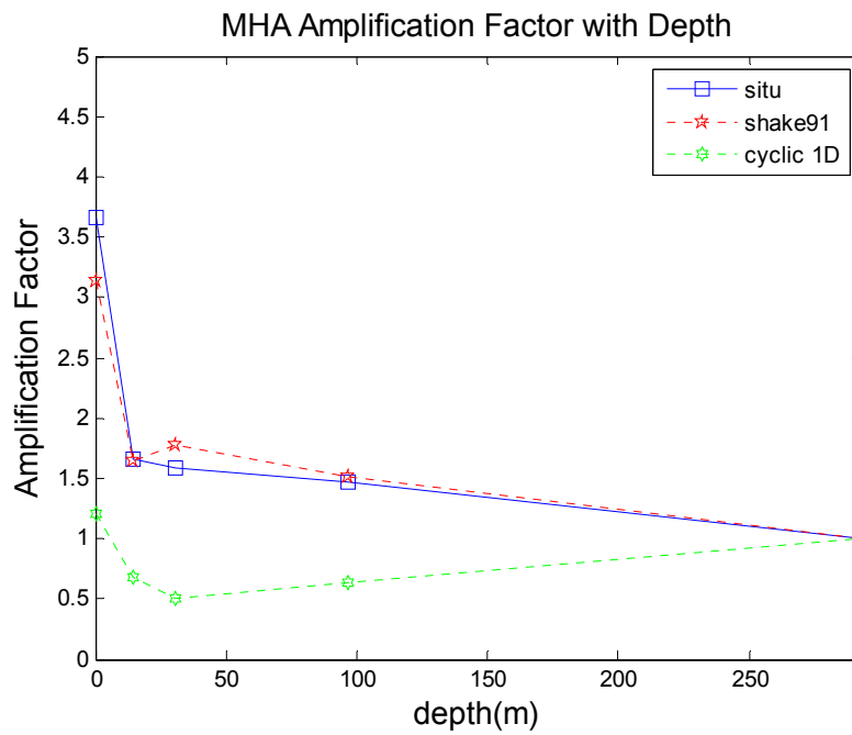
圖 3.36 最大加速度放大係數隨深度變化圖
