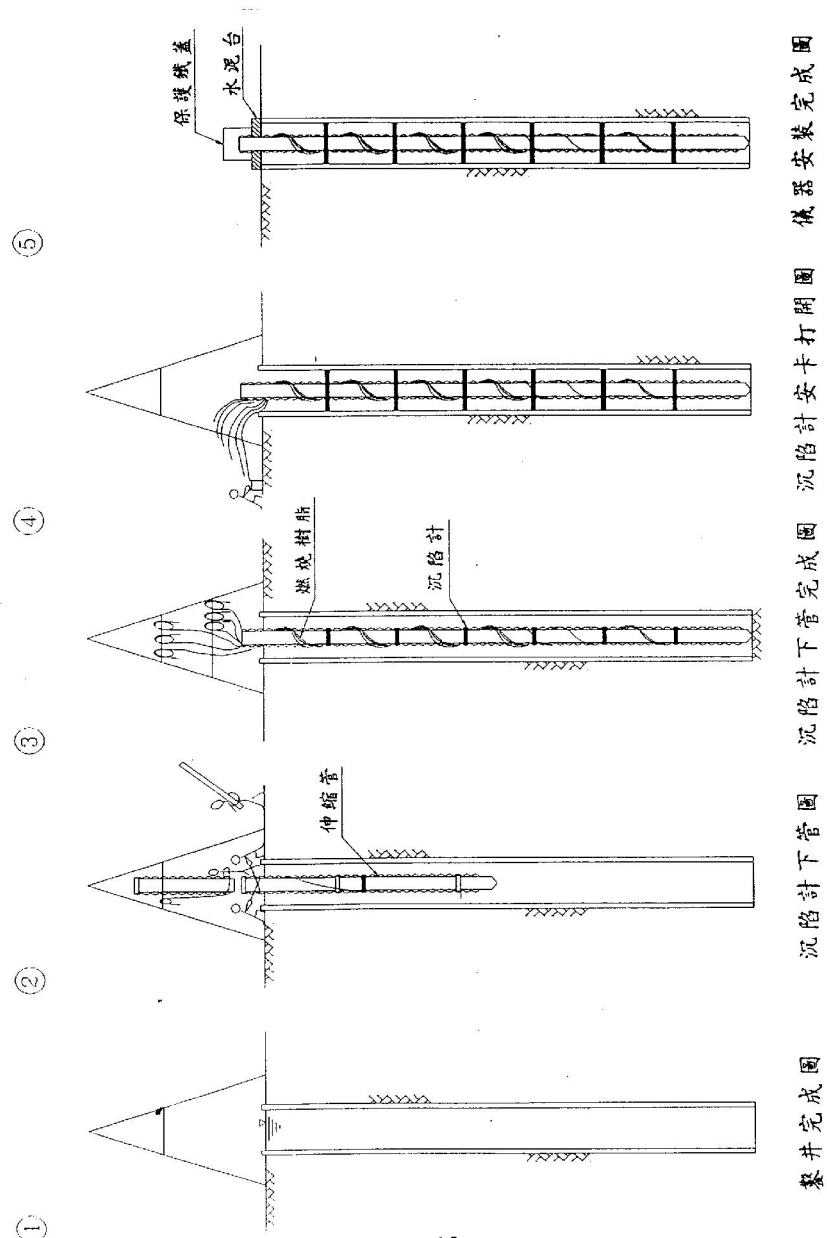
圖 5.4 沉陷計安裝示意圖
