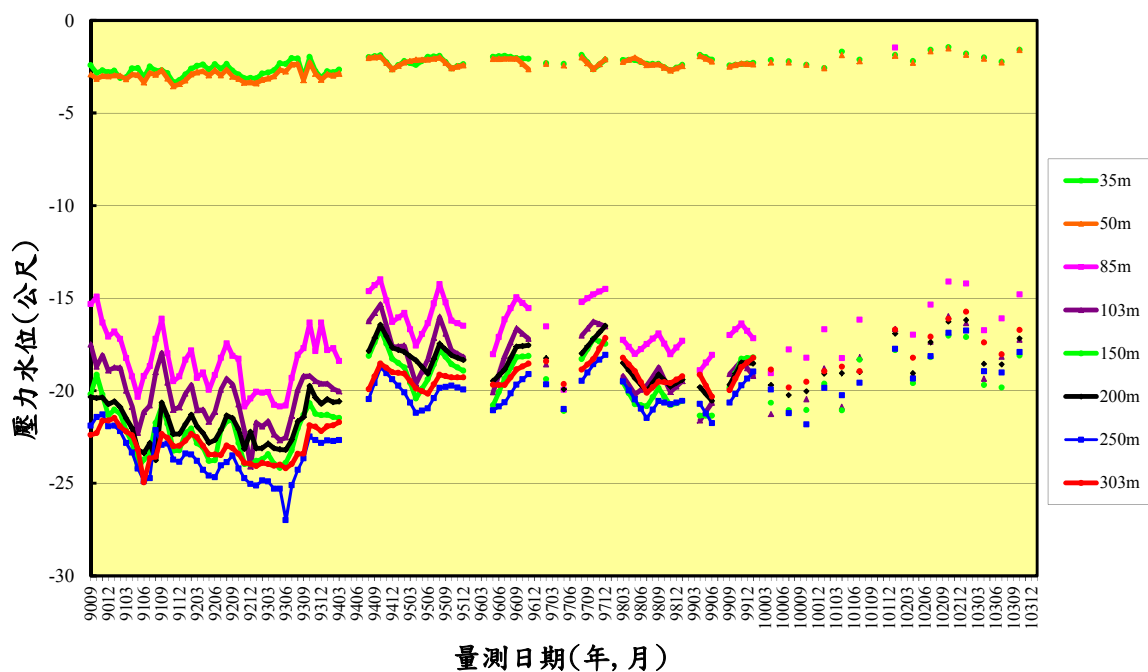
圖 5.9 布袋港(300m)分層水位變化圖(手動量測)
