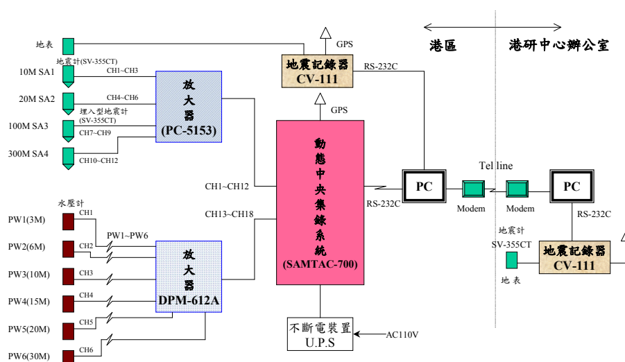
圖 2.1 港區地震監測系統規劃與流程圖
