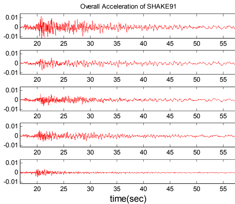
圖 3.35b 各深度加速度歷時比較圖(Shake91)
