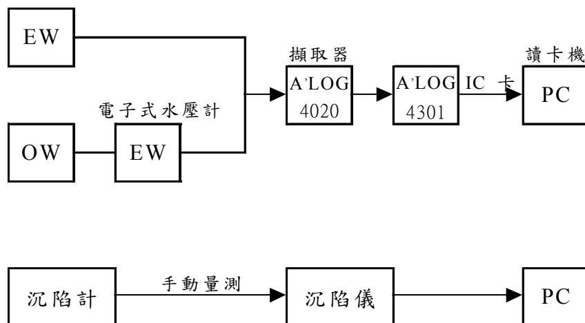
圖 2.15 系統儀器架構流程圖
