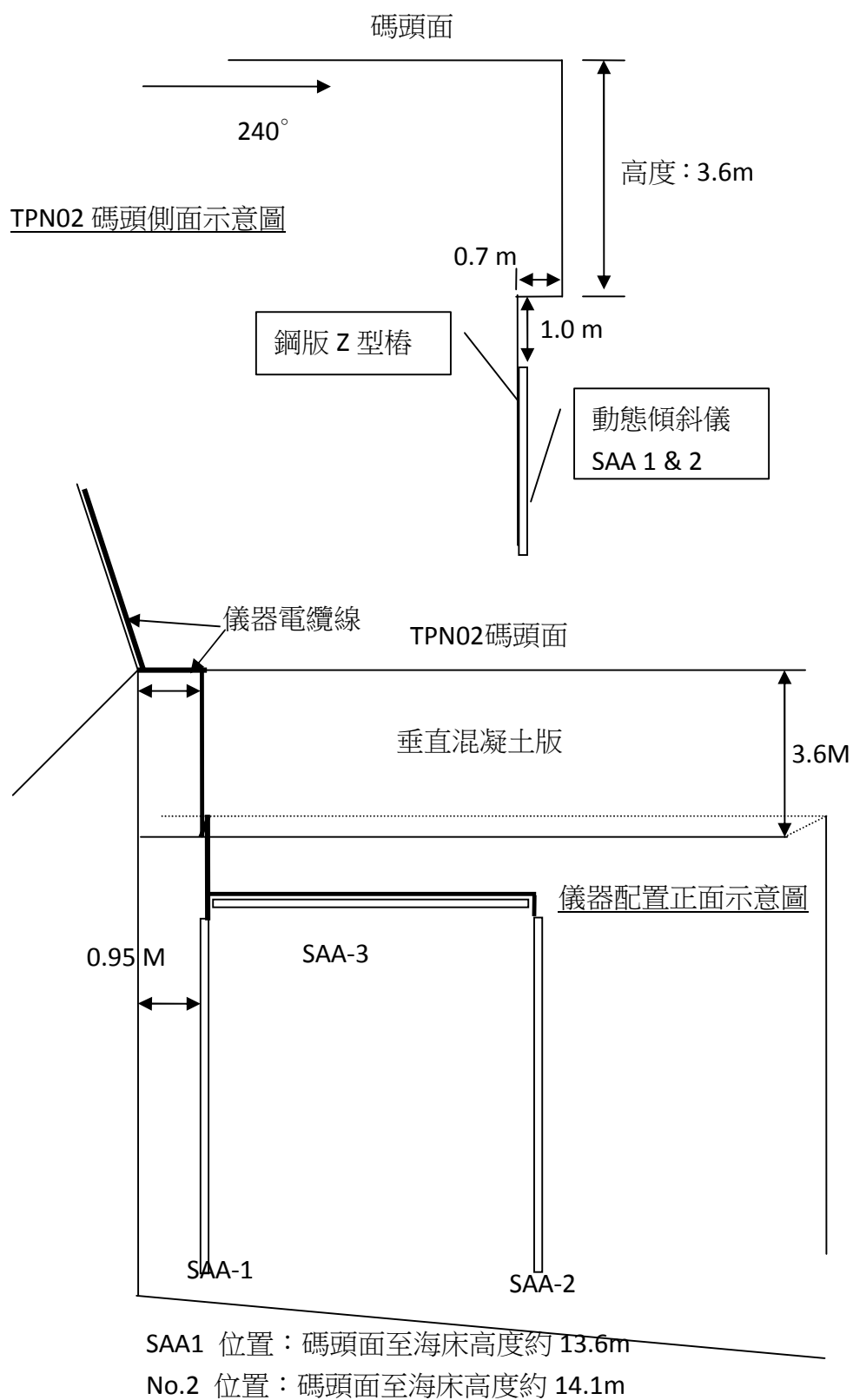
圖 4.17 TPN02 板樁變位監測配置圖
