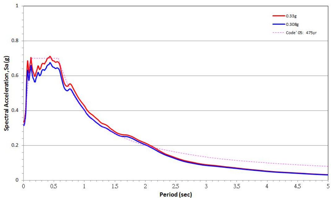
圖 3.15c 安平港 A、B 類型地震水平加速度反應譜曲線圖(0.308g、0.33g)
