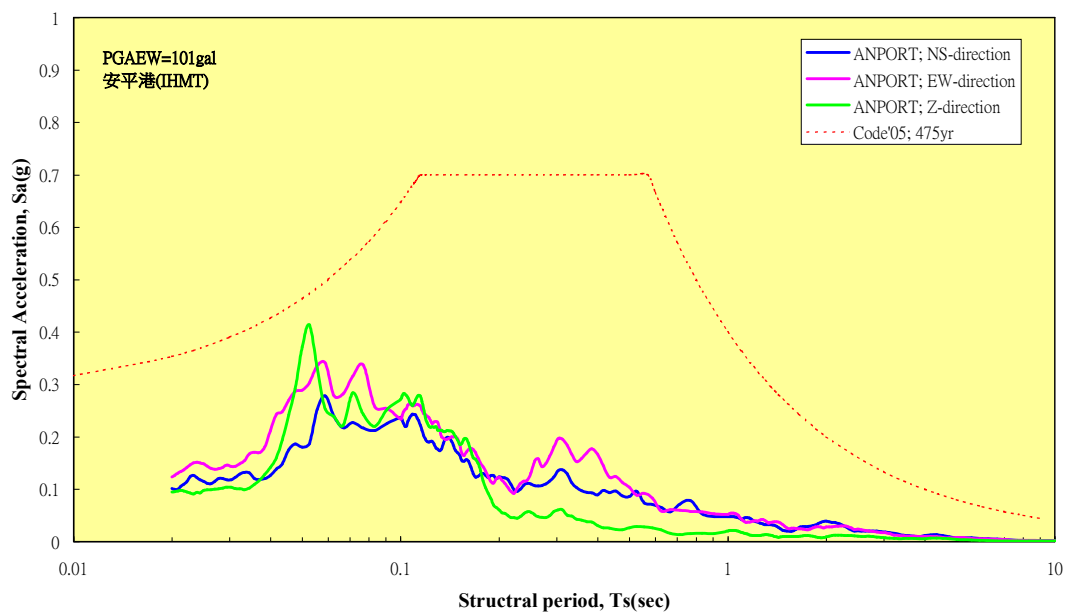
圖 3.49 安平港地震站實測加速度反應譜圖(港研中心) ( \zeta=5\% )
