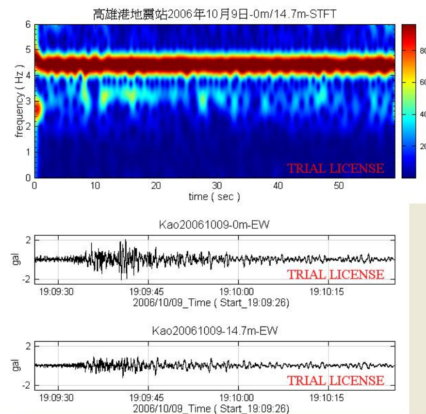
圖 3.60 高雄港地震站 2006 年 10 月 9 日地震 STFT 法頻譜比圖
