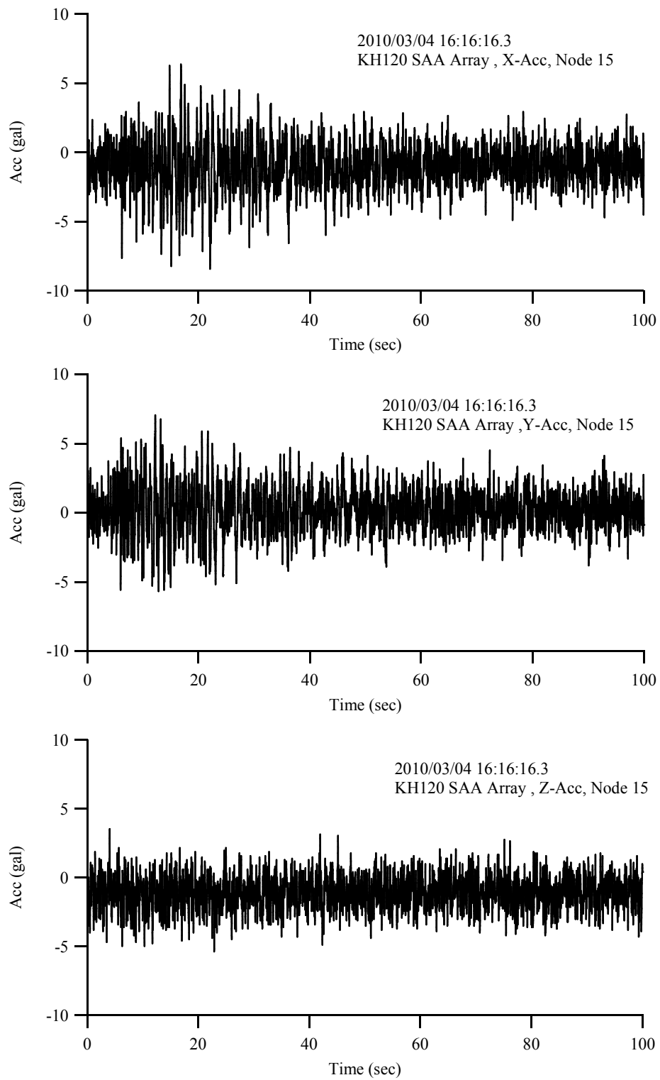
圖 4.5 KH120 之 SAA 頂端加速度歷時
