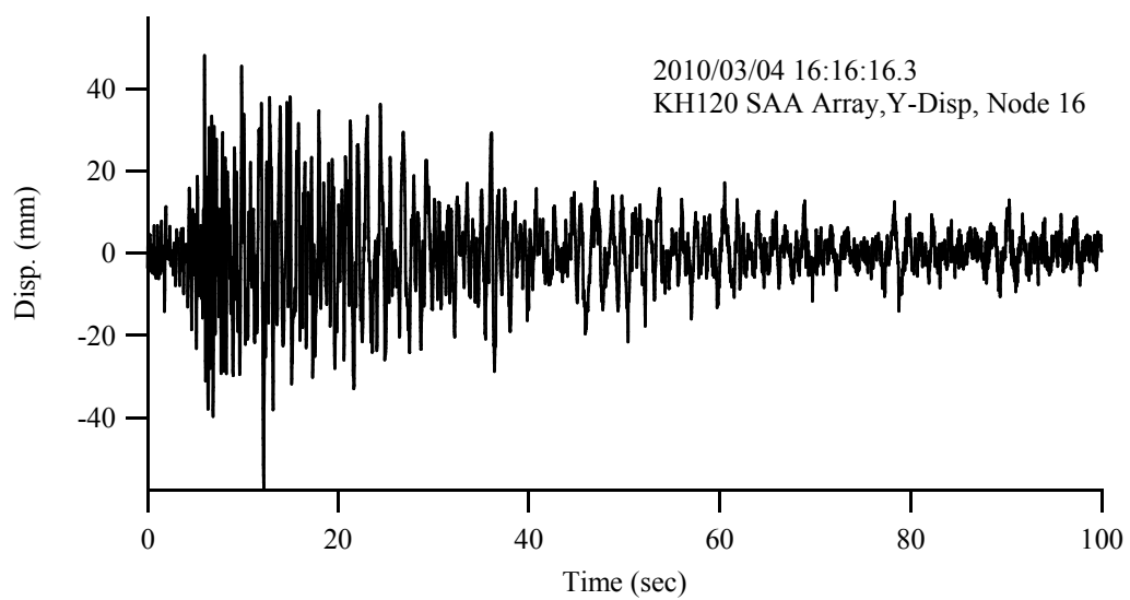
圖 4.6 KH120 SAA 頂端位移歷時
