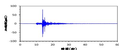
圖 3.12c 安平港 C 類型地震歷時圖
