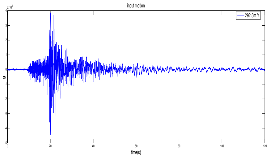
圖 3.29 地震輸入運動(292.5 公尺 Y 向)
