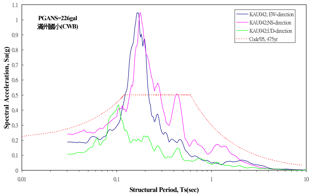
圖 3.42 滿州國小(KAU042)地震站實測反應譜圖(中央氣象局)
