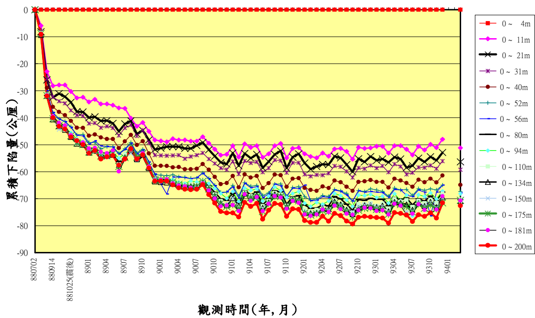
圖 5.25 安平港分層累積下陷量圖
