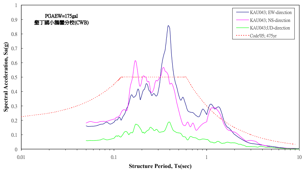
圖 3.43 墾丁國小(KAU043)地震站實測反應譜圖(中央氣象局)
