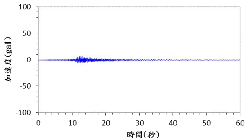
圖 3.12a 安平港 A 類型地震歷時圖
