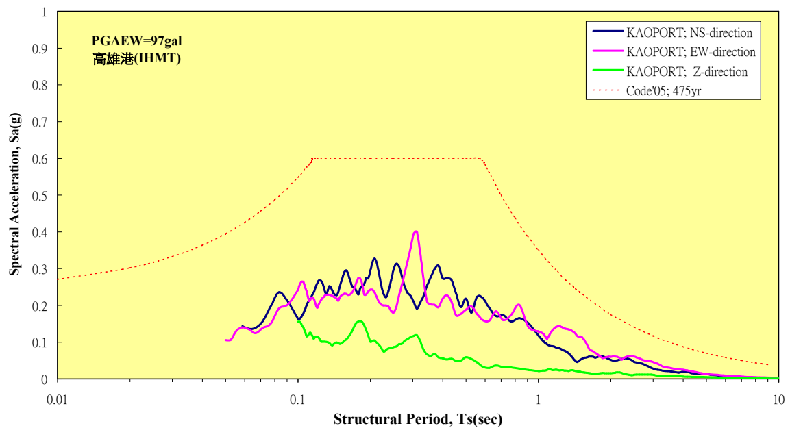
圖 3.47 高雄港地震站實測加速度反應譜圖( \zeta=5\% ) (港研中心)
