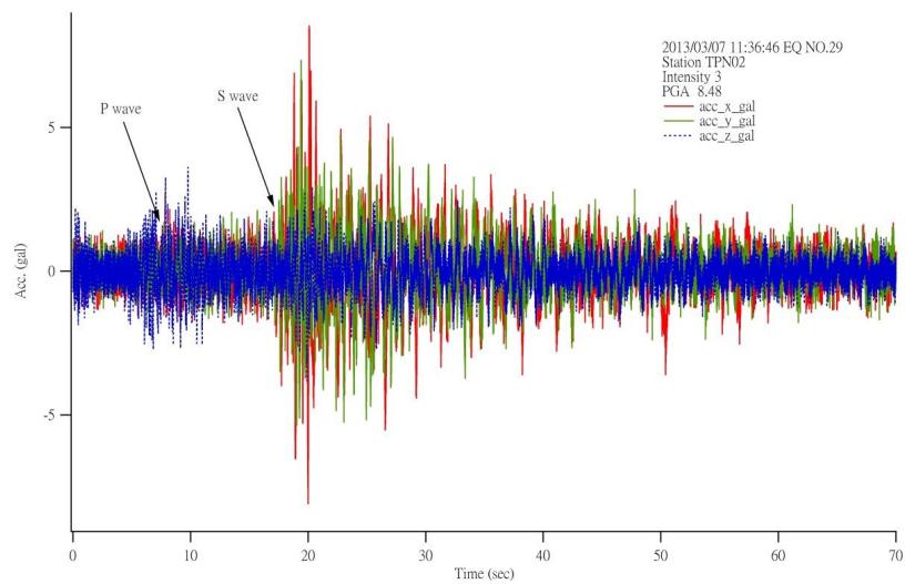
圖 4.19 2013/03/07 TPN02 監測站地表加速度計歷時
