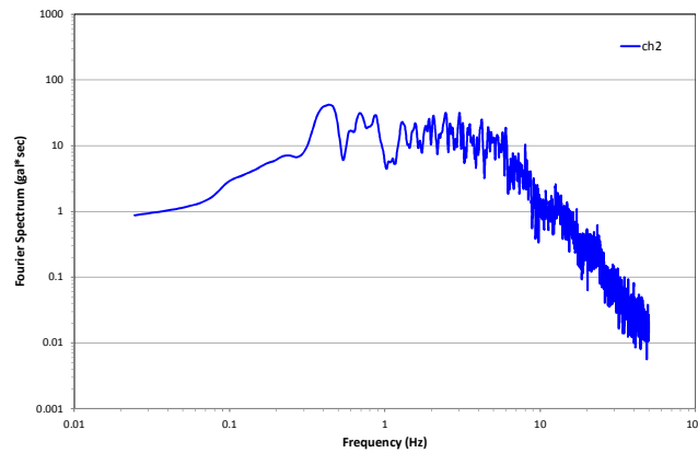
圖 3.19b 臺中港 B 類型地震加速度富氏譜圖
