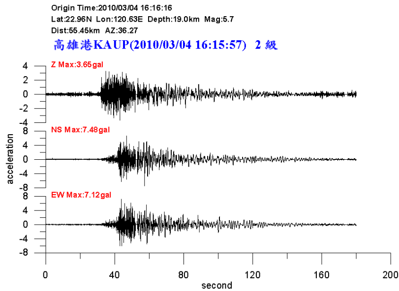
圖 4.3 高雄港監測站加速度歷時(氣象局)
