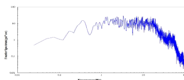
圖 3.13b 安平港 B 類型地震加速度富氏譜圖
