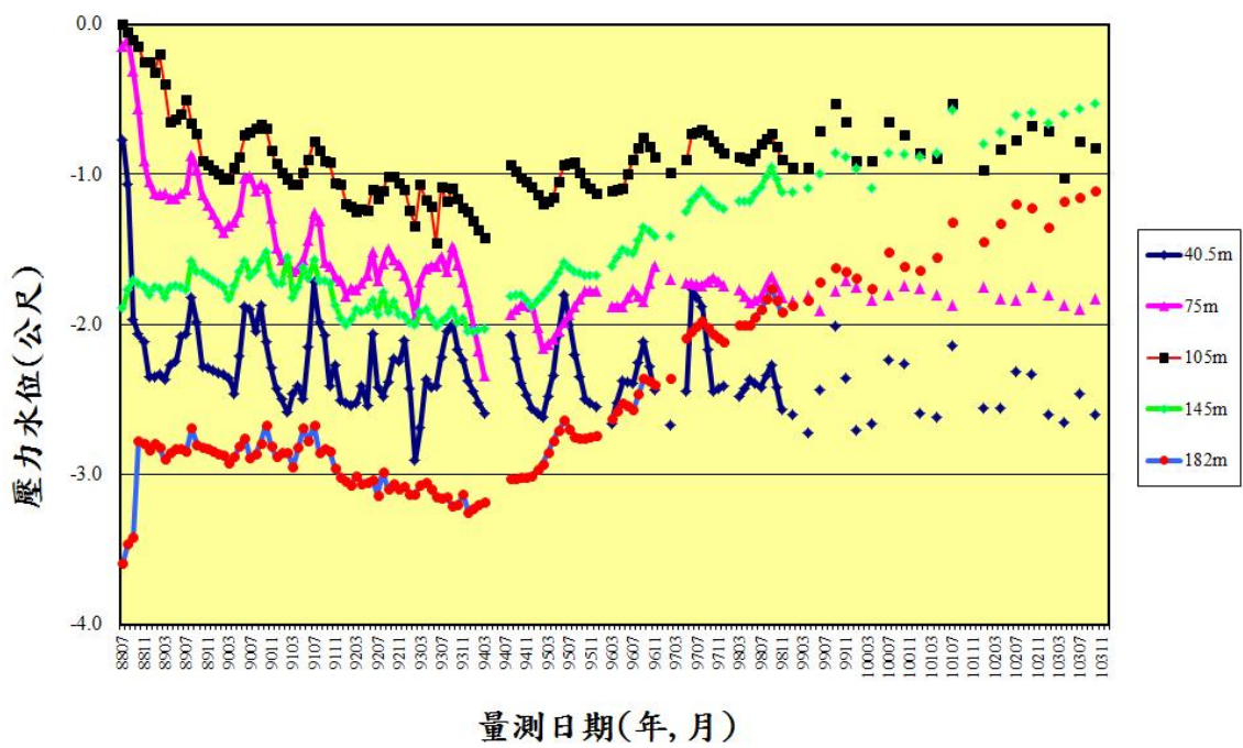
圖 5.24 安平港分層水位變化圖(手動量測)
