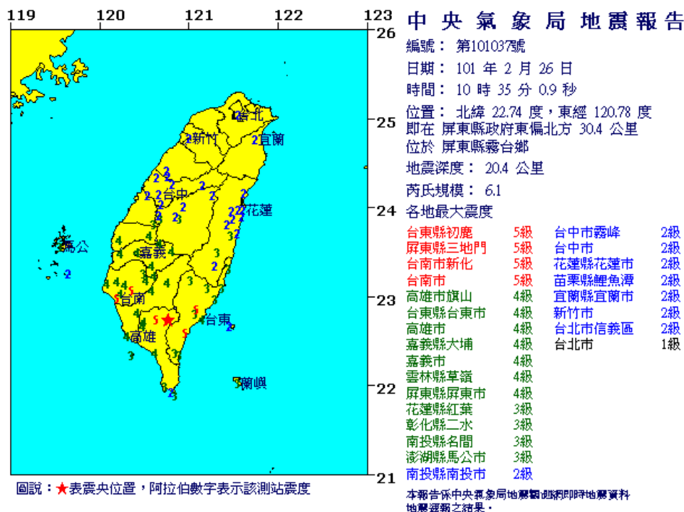
圖 3.52 2012 年 02 月 26 日地震震度分布(中央氣象局)
