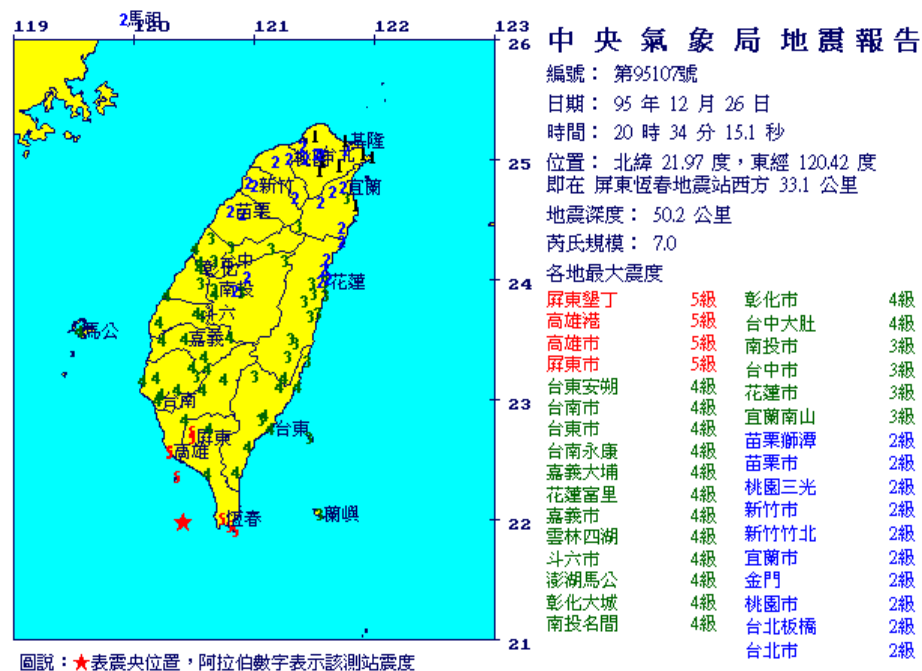
圖 3.50 2006 年 12 月 26 日恆春地震震度分布(中央氣象局)
