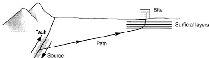
圖 3.22 地震波傳遞示意圖
