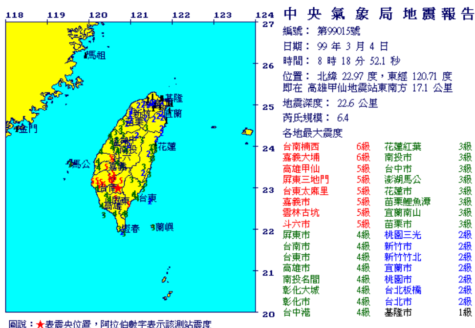
圖 3.51 2010 年 03 月 04 日甲仙地震震度分布(中央氣象局)
