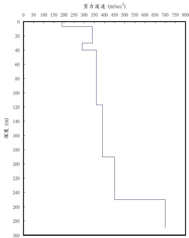
圖 3.27 高雄港地震監測站剪力波速隨深度變化圖
