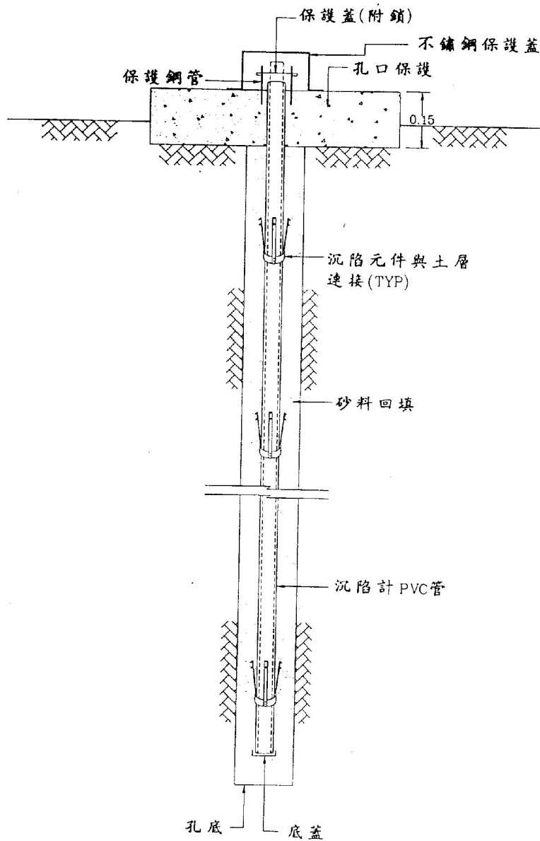
圖 5.5 磁感式層別沉陷計安裝示意圖
