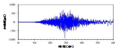
圖 3.12b 安平港 B 類型地震歷時圖
