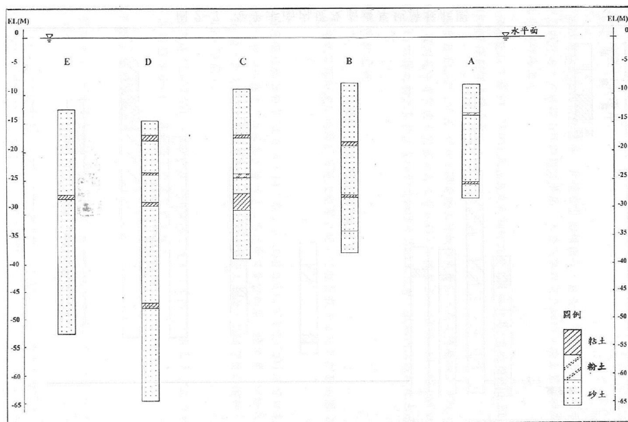
圖 3.8 安平港外防波堤碼頭地層柱狀圖
