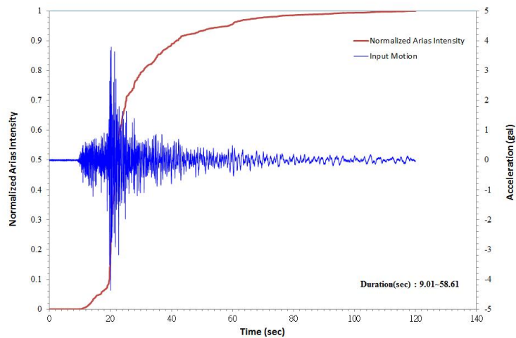
圖 3.30 輸入地震延時
