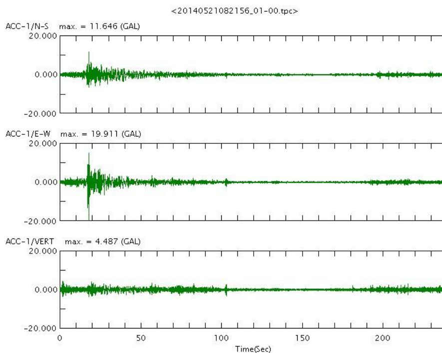
圖 3.38b 臺中港區地震即時監測加速度歷時圖
