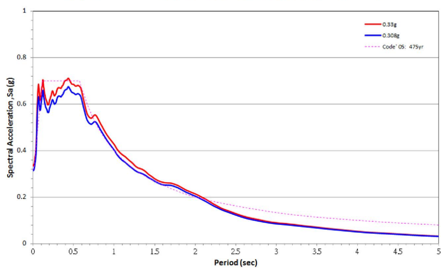
安平港2006~2013地震水平地表加速度反應譜平均圖(阻尼比=5%)
