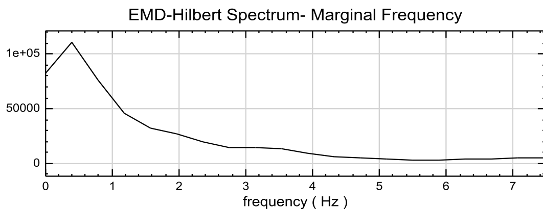
圖 3.59 高雄港地震站 2006 年 12 月 26 日恆春地震能譜圖
