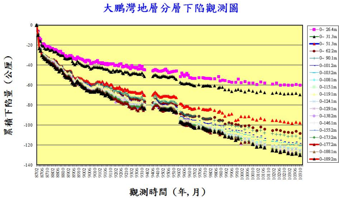
圖 5.21 大鵬灣地層分層下陷觀測圖
