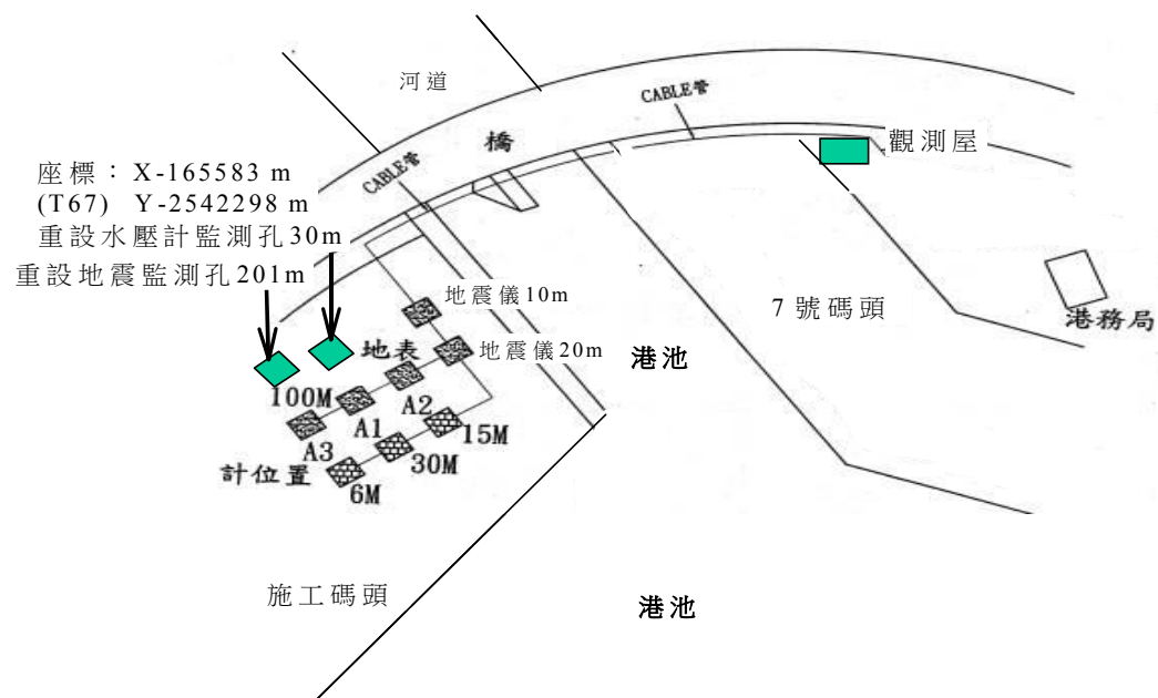
圖 2.5 安平港區井下地震監測站平面示意圖
