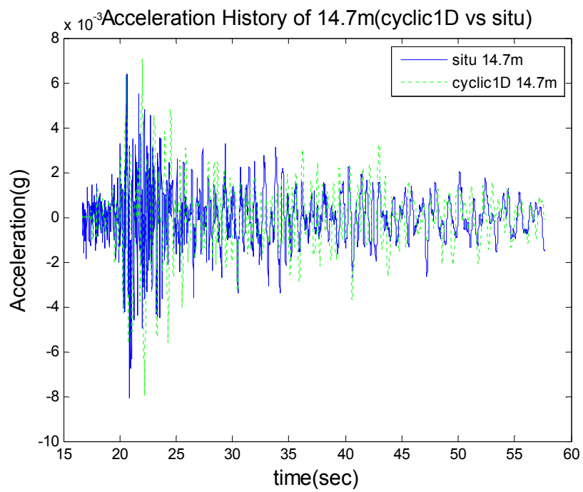
圖 3.33b 現地與 Cyclic1D 加速度歷時比較圖(-14.7m)
