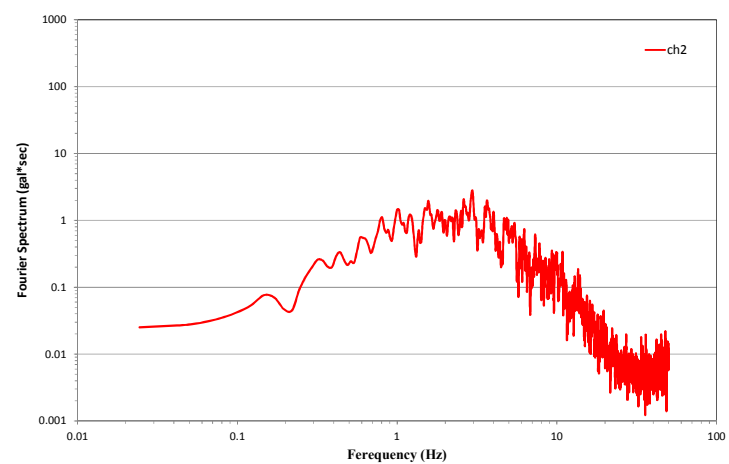
圖 3.19a 臺中港 A 類型地震加速度富氏譜圖
