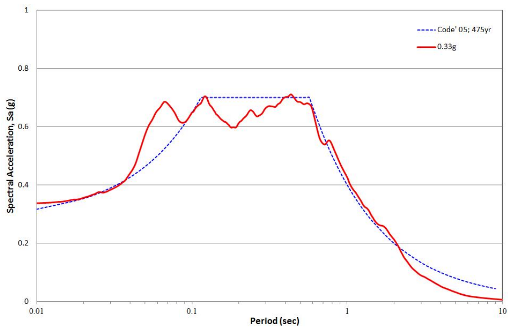
圖 3.15b 安平港 A、B 類型地表地震水平加速度反應譜曲線圖(0.33g)
