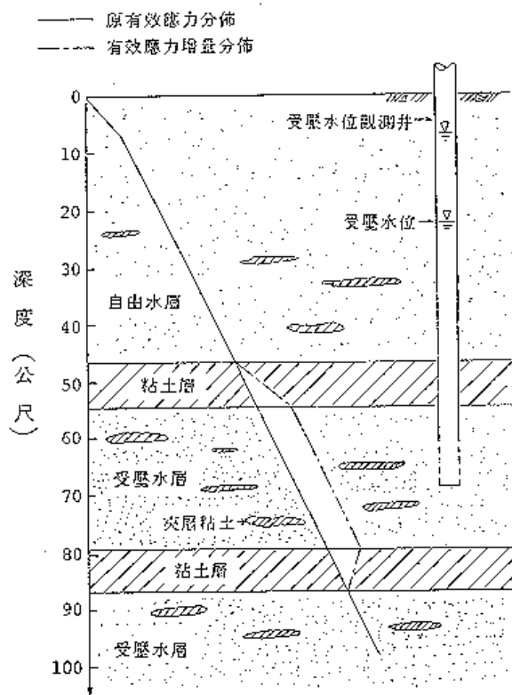
圖 5.3 受壓水位下降引致之有效應力增量分布
