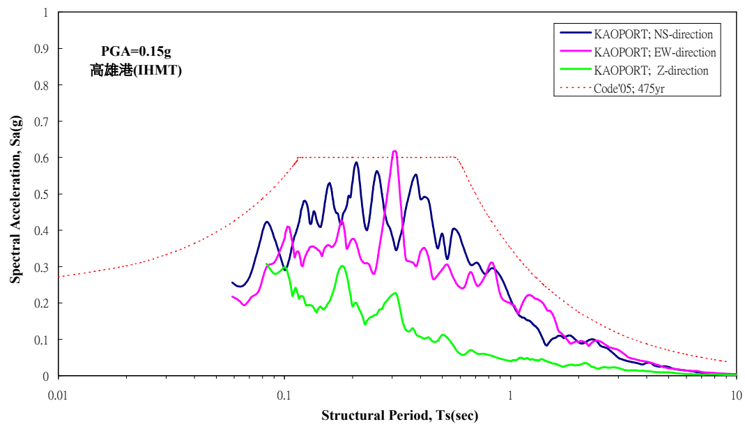
圖 3.48 高雄港地震站加速度反應譜圖(0.15g) (港研中心)
