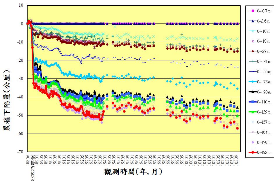
圖 5.23 臺中港分層累積下陷量圖(200m)
