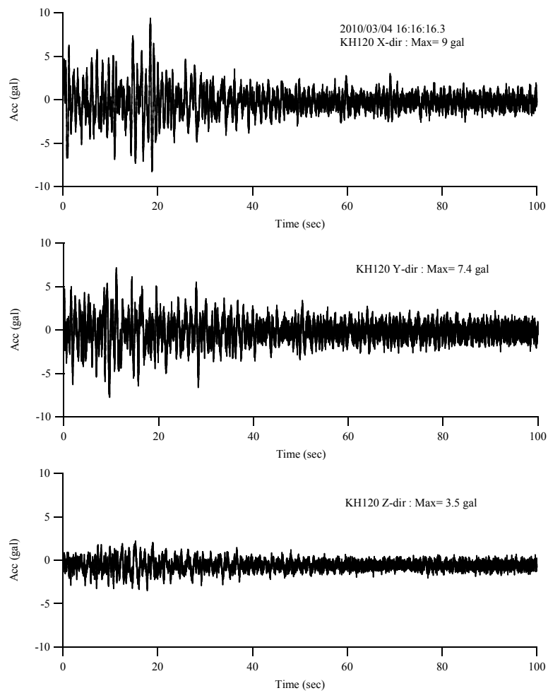
圖 4.4 KH120 水下地震儀記錄
