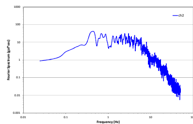
臺中港B類型地震加速度富氏譜圖
