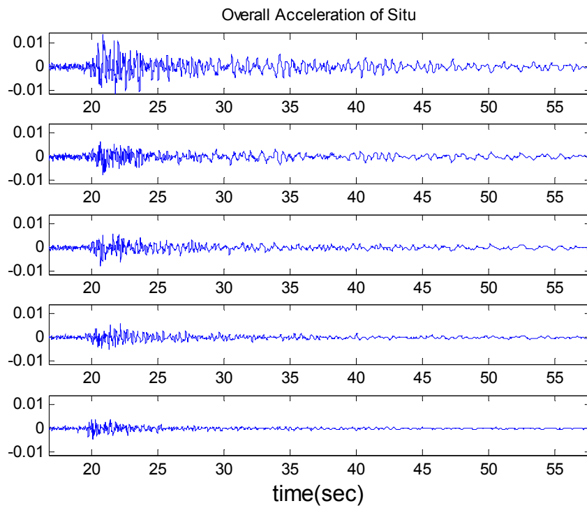
圖 3.35c 各深度加速度歷時比較圖(現地)
