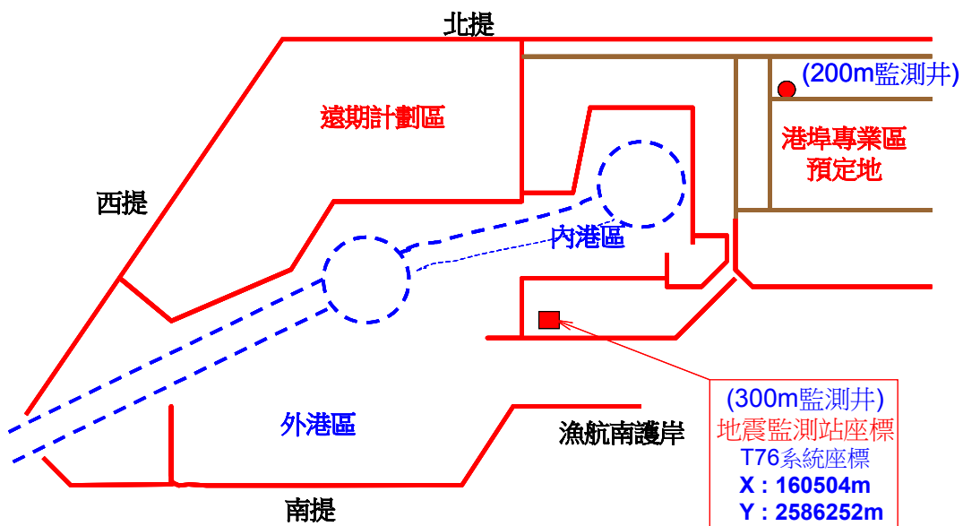
圖 2.8 布袋港區井下地震監測站平面示意圖
