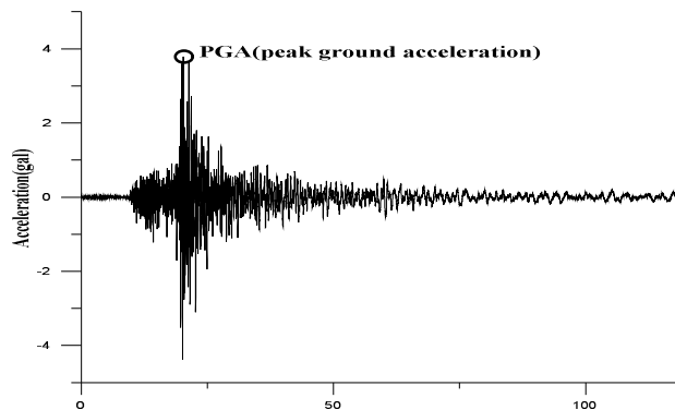
圖 3.31 地震 PGA 示意圖
