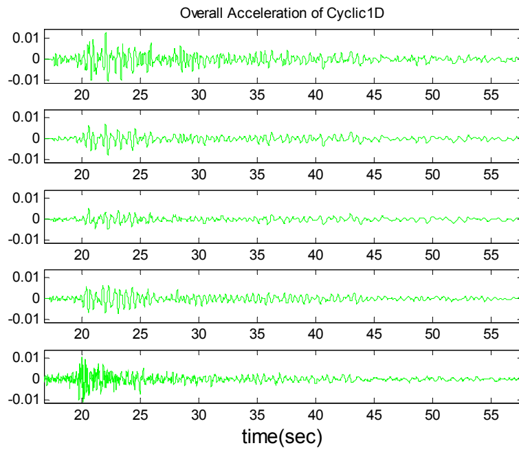
圖 3.35a 各深度加速度歷時比較圖(Cyclic1D)
