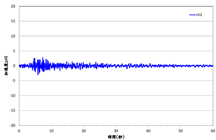
圖 3.18a 臺中港 A 類型地震歷時圖
