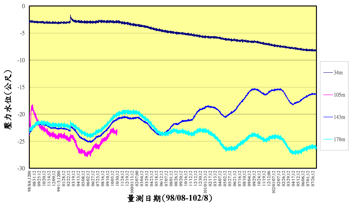
圖 5.7b 布袋港分層水位變化圖(自記式)
