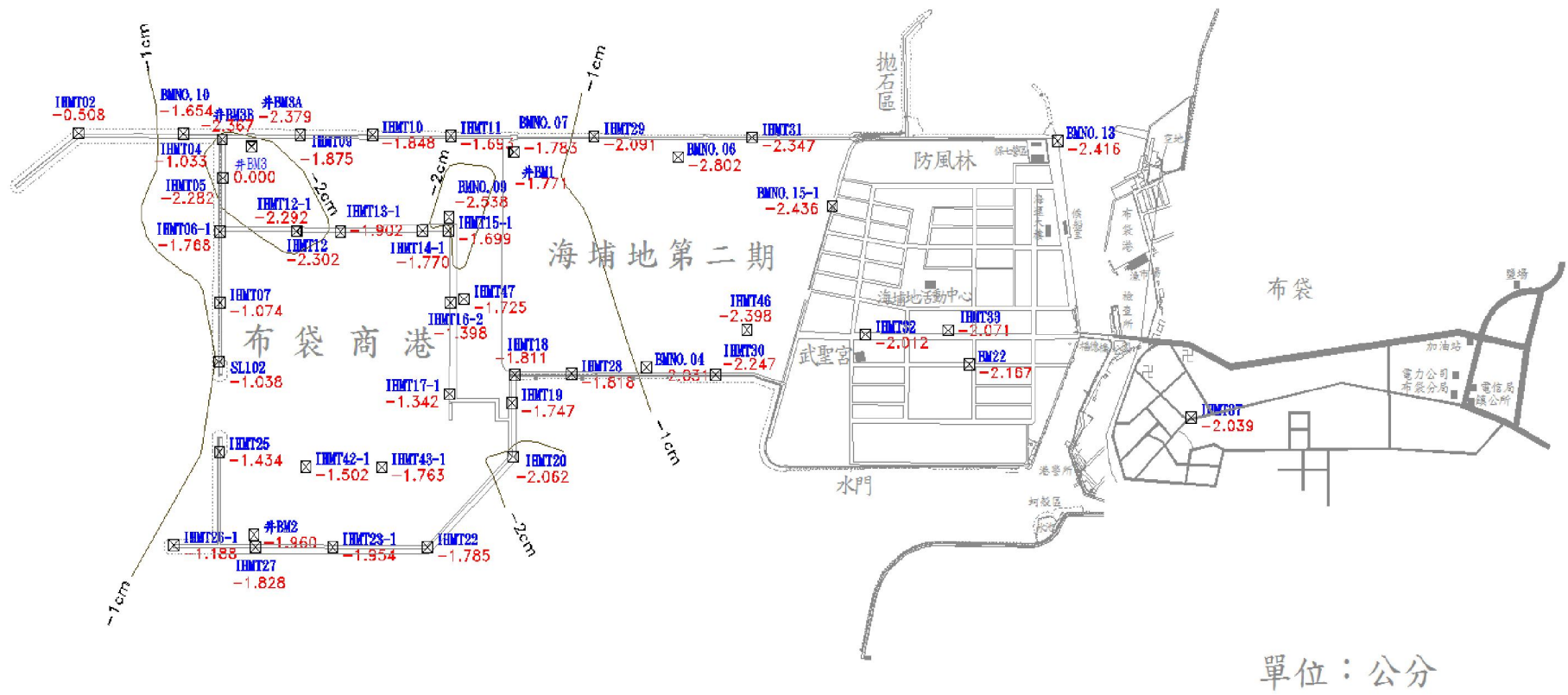
圖 5.19 嘉義縣布袋鎮及布袋港區下陷圖(102~103 年)
