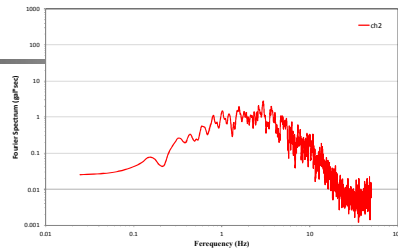
臺中港A類型地震加速度富氏譜圖
