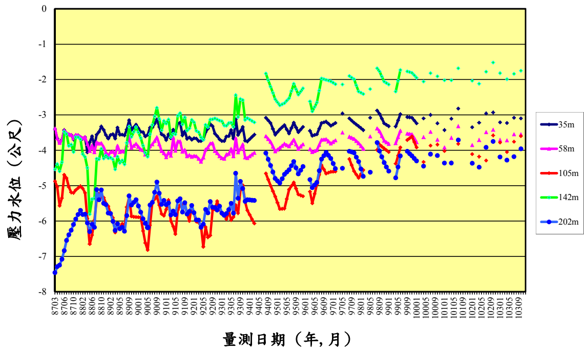
圖 5.20 大鵬灣分層水位變化圖(手動量測)
