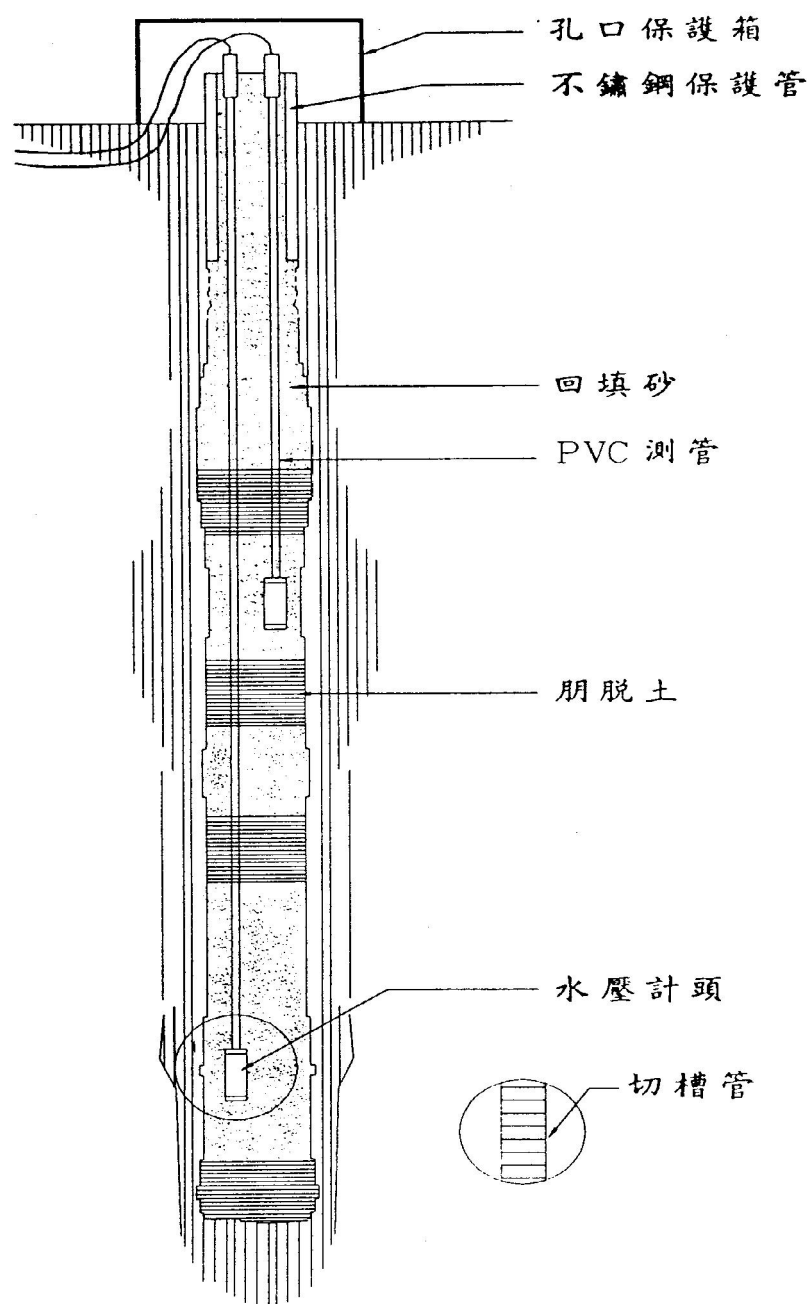
圖 2.17 開放式水壓計安裝示意圖
