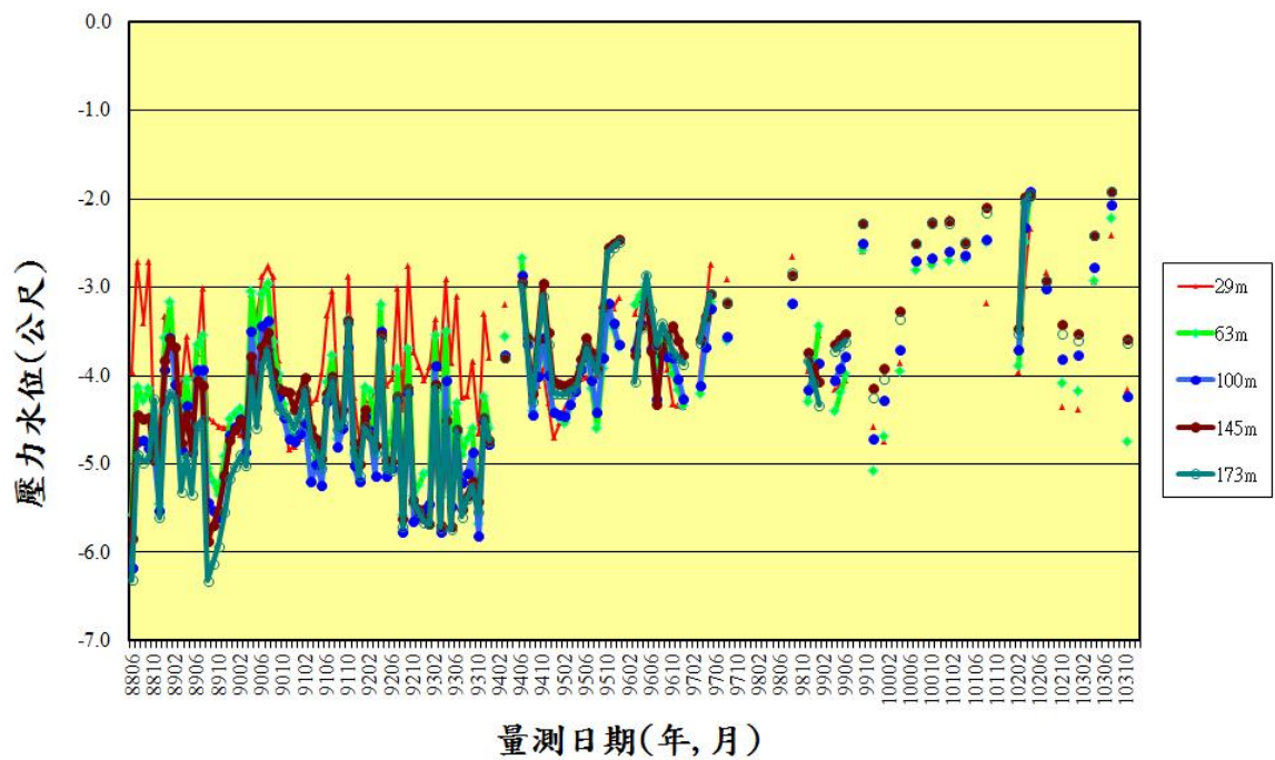
圖 5.22 臺中港分層水位變化圖(手動量測)
