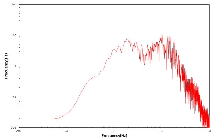
圖 3.13c 安平港 C 類型地震加速度富氏譜圖
