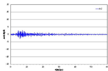
臺中港 A 類型地震歷時圖
