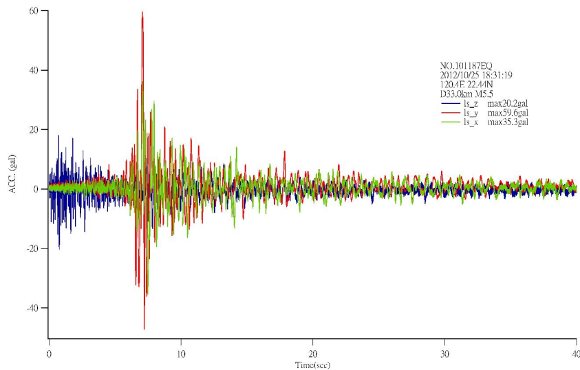
圖 4.10 2012/12/15 KH120 陸上地震儀記錄
