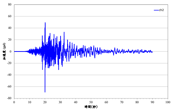
圖 3.18b 臺中港 B 類型地震歷時
