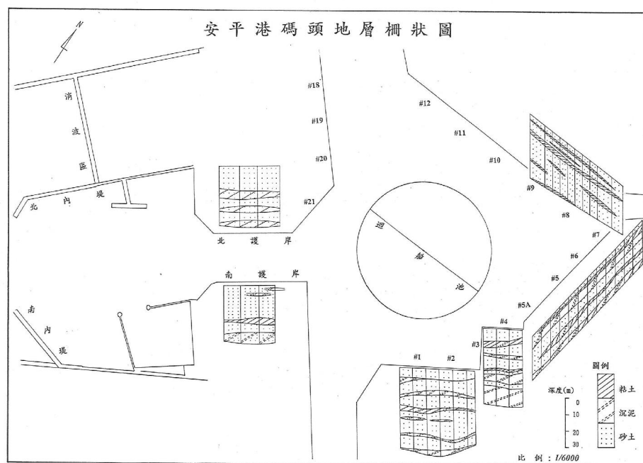
圖 3.9 安平港碼頭地層柵狀圖
