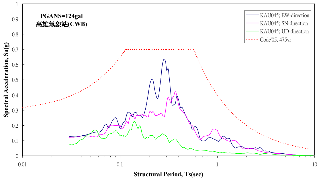
圖 3.45 高雄氣象地震站實測反應譜圖(中央氣象局)
