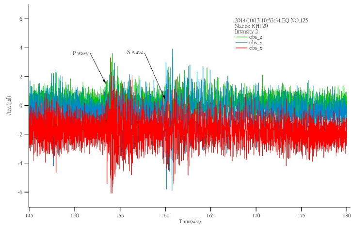
圖 4.12 2014/10/13 KH120 水下地震儀記錄
