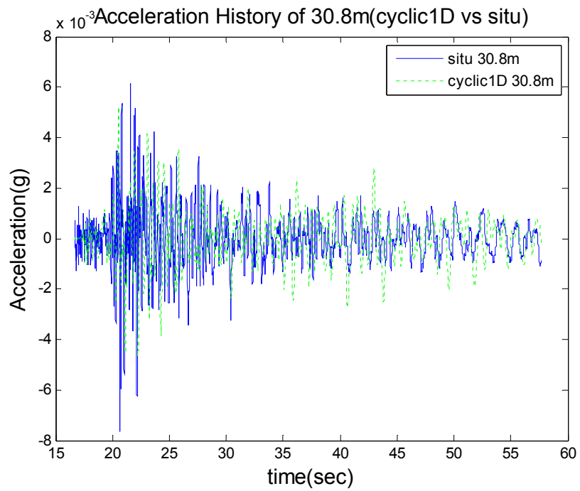
圖 3.33c 現地與 Cyclic1D 加速度歷時比較圖(-30.8m)
