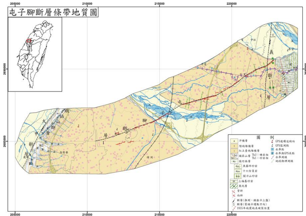
圖 3.16 屯子腳斷層條帶地質圖
