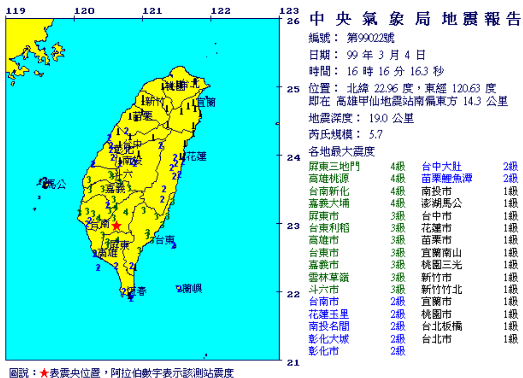
圖 4.2 2010/03/04 甲仙地震震度分佈(氣象局)
