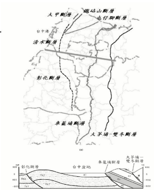
圖 2 台灣中西部地區活動斷層分佈圖。 (a)活動斷層分佈；(b)活動斷層剖面圖(根據中央地質調查所網站資料重繪)
