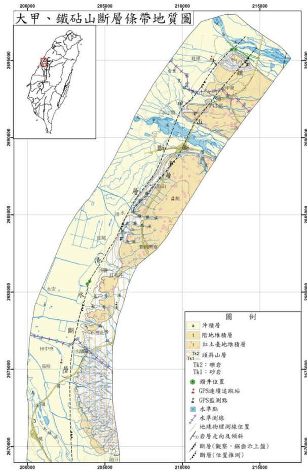
圖 3.17 大甲斷層與鐵砧山斷層條帶地質圖
