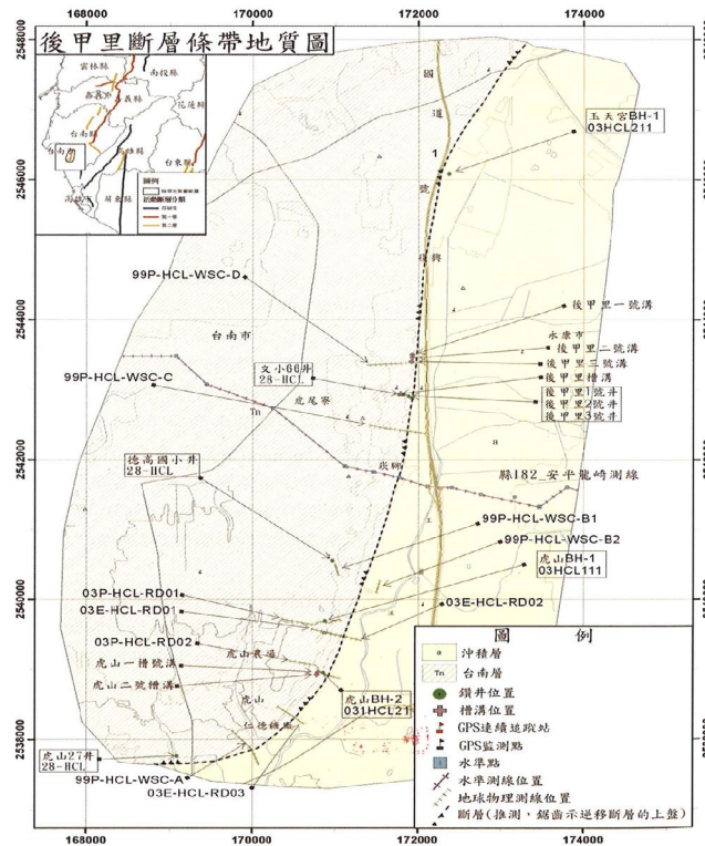
圖 3.11 後甲里斷層地質圖
