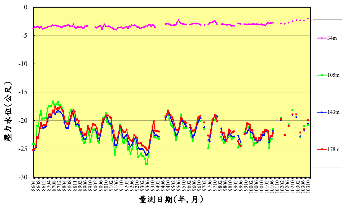
圖 5.8 布袋港(200m)分層水位變化圖(手動量測)
