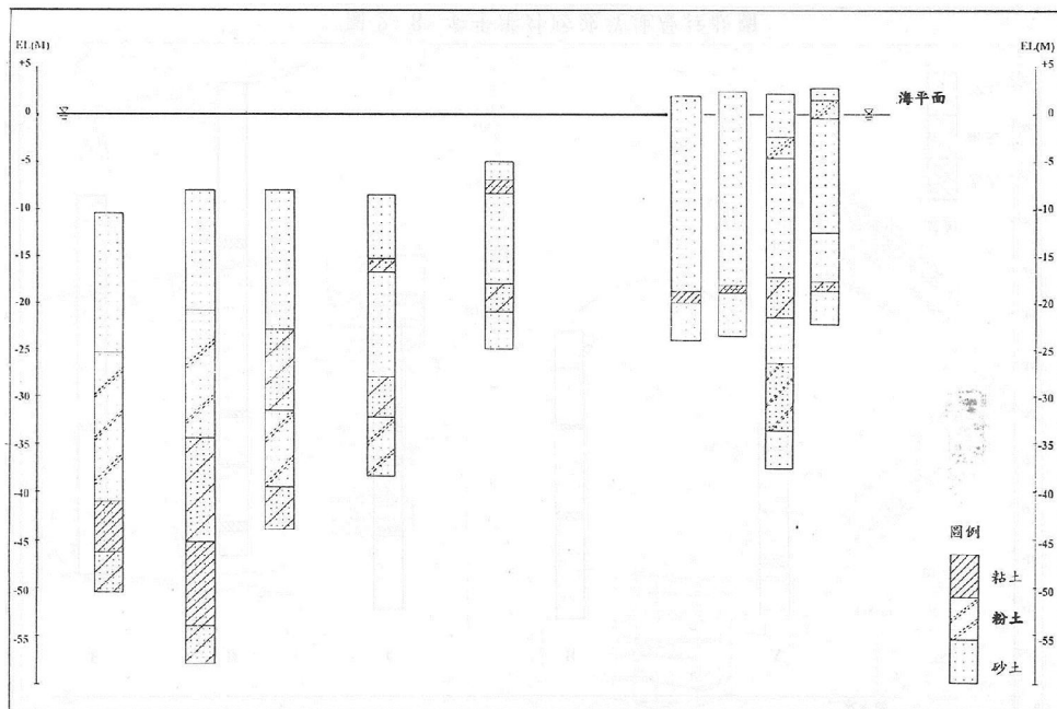
圖 3.7 安平港南內堤、南護岸碼頭地層柱狀圖
