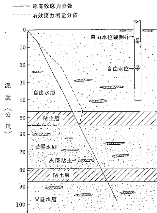
圖 5.2 自由水位下降引致之有效應力增量分布
