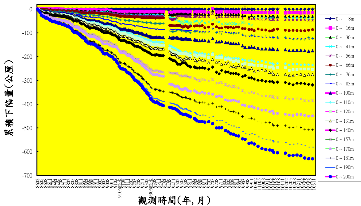
圖 5.10 布袋港(200m)分層累積下陷圖(手動量測)
