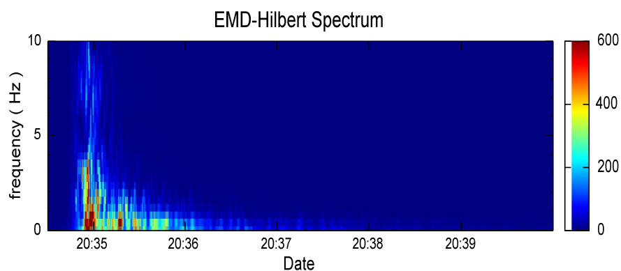
圖 3.58 高雄港地震站 2006 年 12 月 26 日恆春地震(HHT)時頻分析圖
