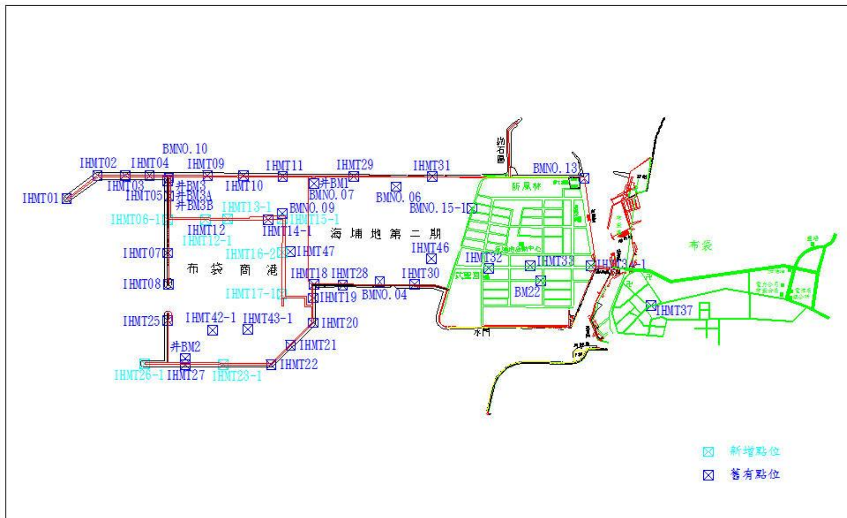
圖 5.13 101 年嘉義縣布袋鎮及布袋港區監測點水準測量工作範圍圖
