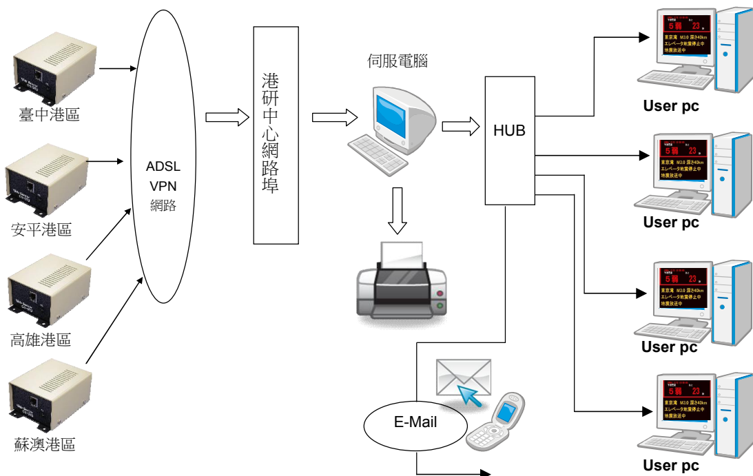
圖 3.37 港區地震災況速報系統儀器配置示意圖
