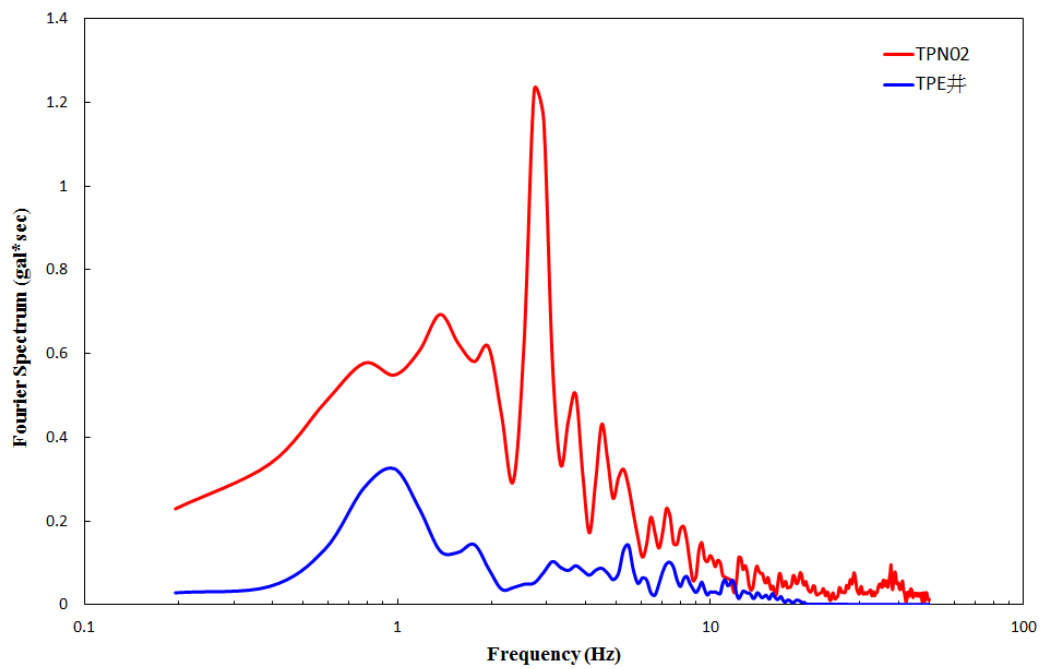
圖 4.23 臺北港北 2 碼頭與井下地震站地表加速度傅式譜比較圖
