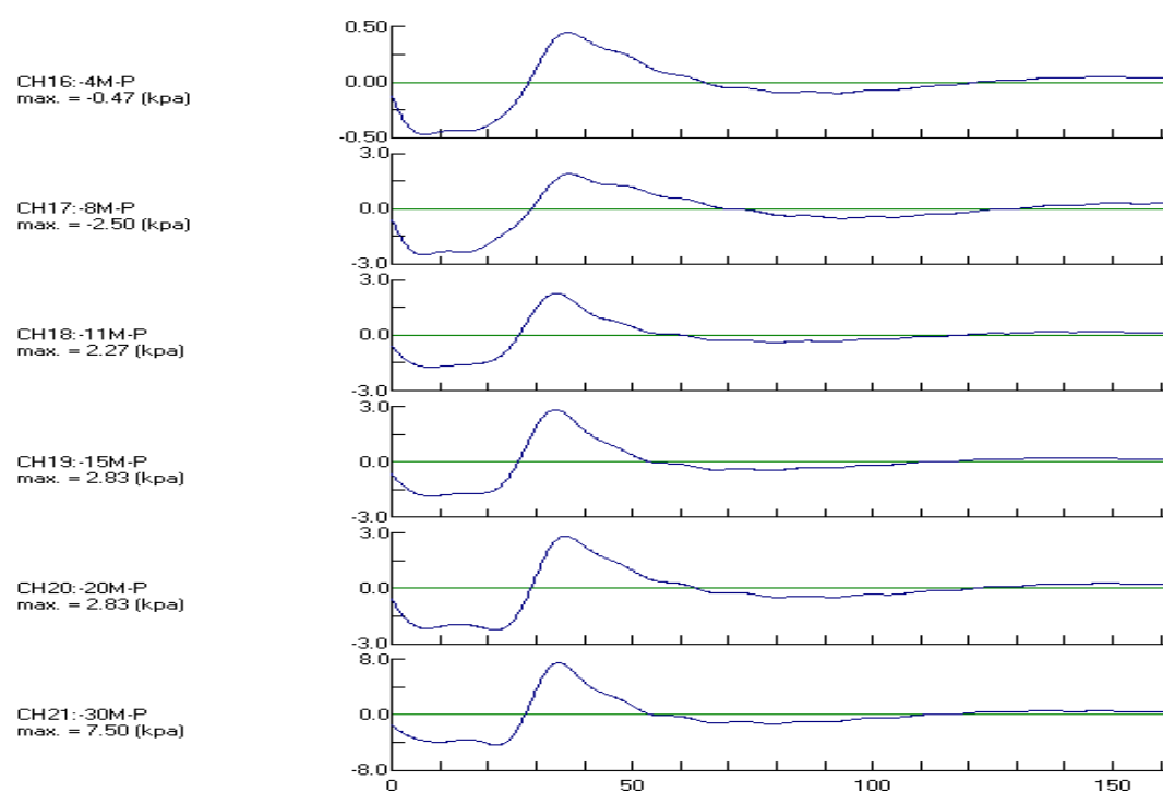
圖 3.54c 安平港 2010 年 3 月 4 日地震之動態孔隙水壓變化 (小於 0.08Hz)
