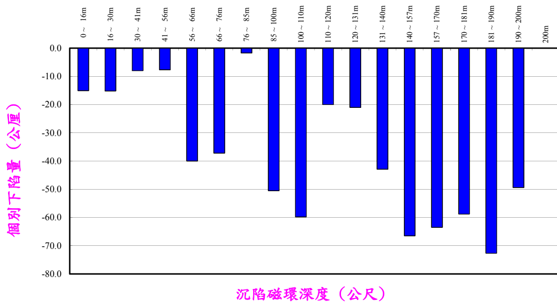
圖 5.11 布袋港(300m)分層個別下陷量圖
