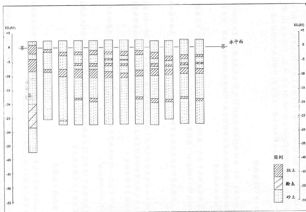
圖 3.5 安平港 8、9、10 號碼頭地層柱狀圖
