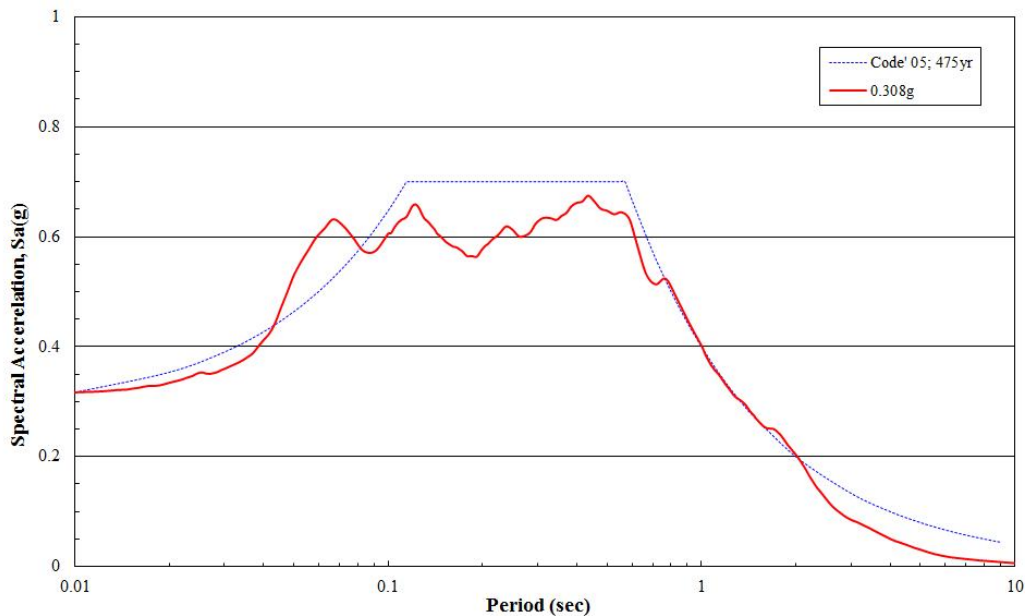
圖 3.15a 安平港 A、B 類型地表地震水平加速度反應譜曲線圖(0.308g)
