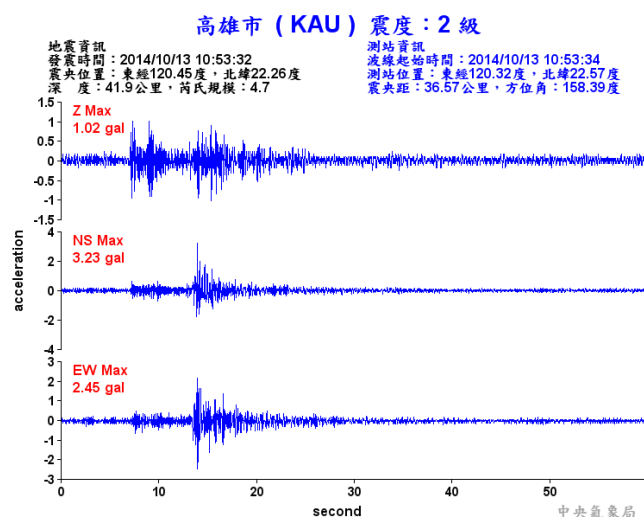
圖 4.11 2014/10/13 高雄市監測站加速度歷時(氣象局)
