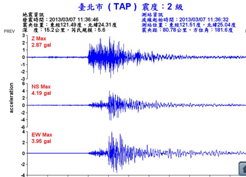
圖 4.18 2013/03/07 臺北市站加速度歷時(氣象局)
