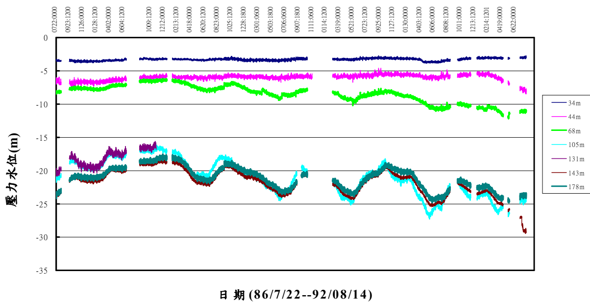
圖 5.7a 布袋港分層水位變化圖(自記式)
