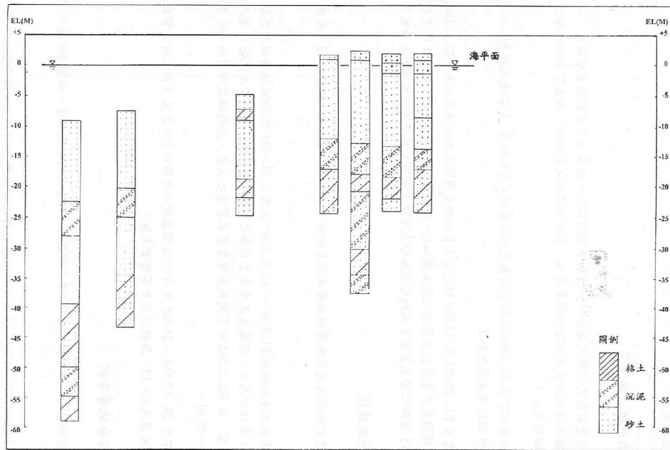
圖 3.6 安平港北內堤、北護岸碼頭地層柱狀圖
