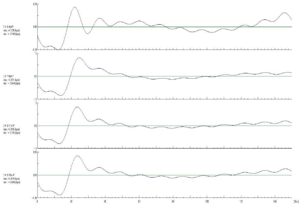
圖 3.55c 安平港 2012 年 2 月 26 日地震之動態孔隙水壓變化 (小於 0.08Hz)
