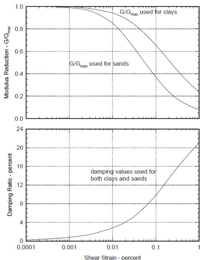
圖 3.28 輸入之剪力模數和阻尼比(SHAKE91)
