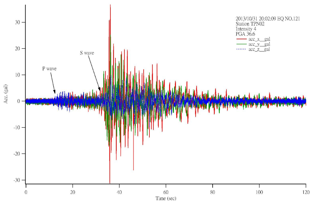
圖 4.21 2013/10/31 TPN02 監測站地表加速度計歷時
