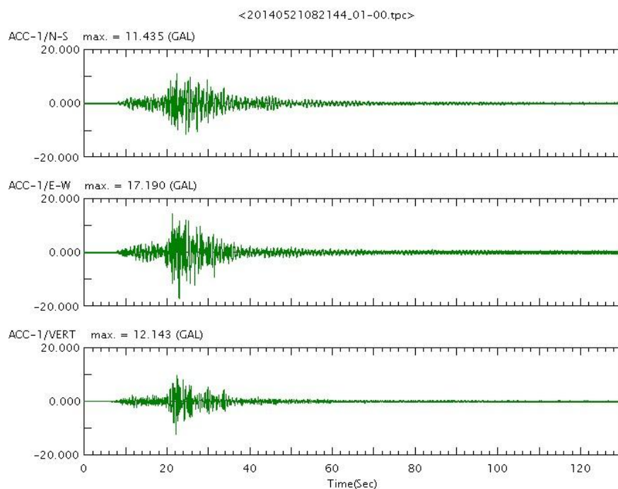
圖 3.41b 蘇澳港區地震即時監測加速度歷時圖
