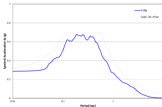
圖 3.20 臺中港地表地震水平加速度反應譜曲線圖(0.28g)
