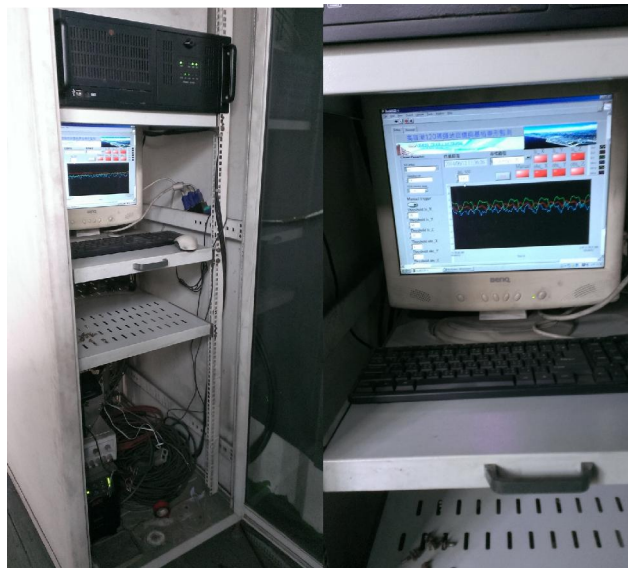
圖 4.14 高雄港 120 號碼頭動態監測站機房(2014/10/25 照)
