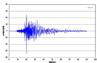
臺中港 B 類型地震歷時
