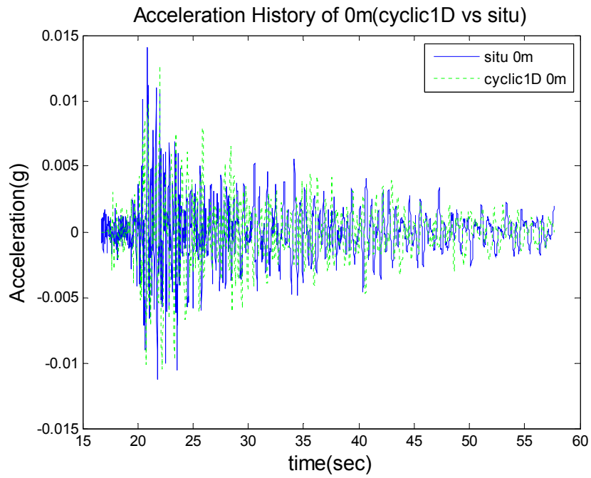
圖 3.33a 現地與 Cyclic1D 加速度歷時比較圖(地表)
