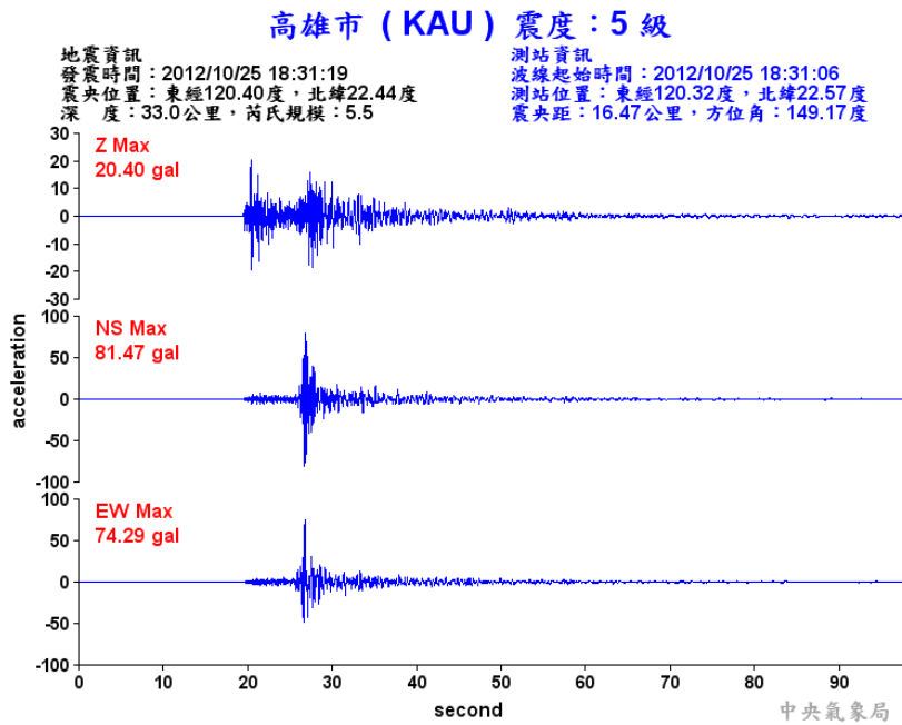
圖 4.8 2012/10/25 高雄港監測站加速度歷時(氣象局)
