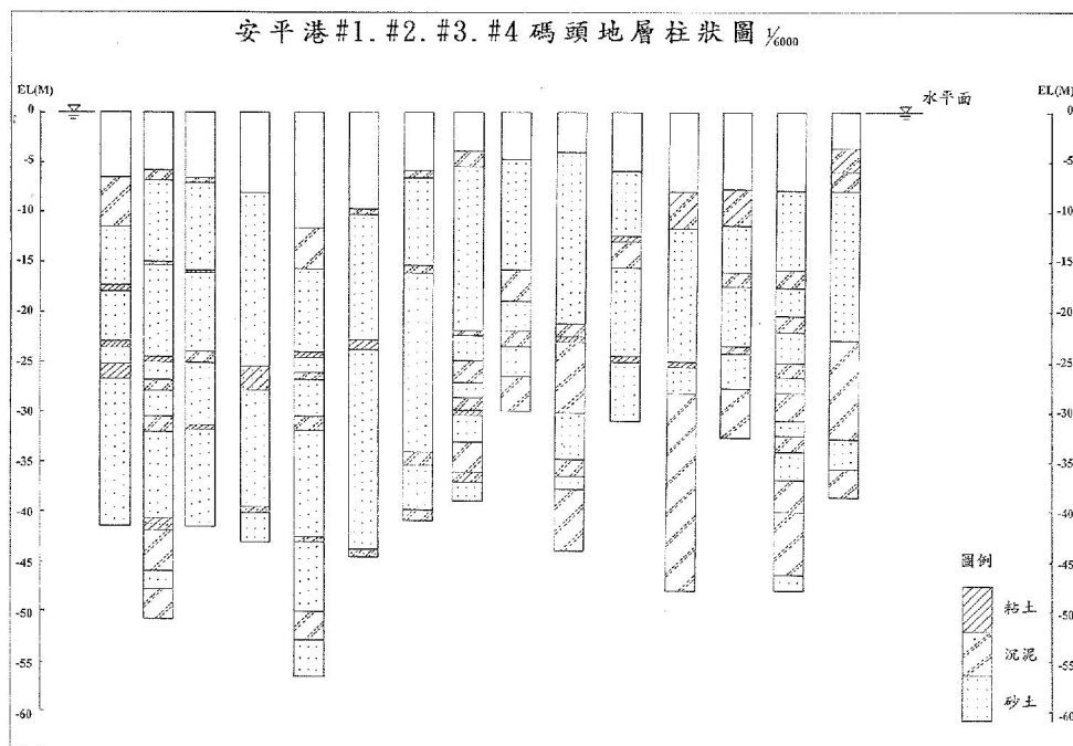
圖 3.3 安平港 1、2、3、4 號碼頭地層柱狀圖
