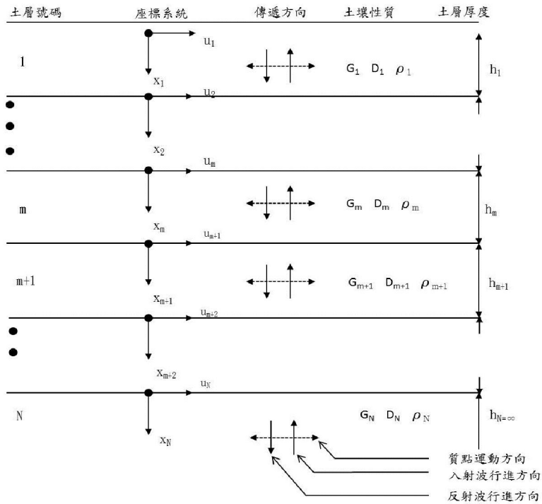
圖 3.23 一維土層系統剖面(Schnabel et al.,1972)
