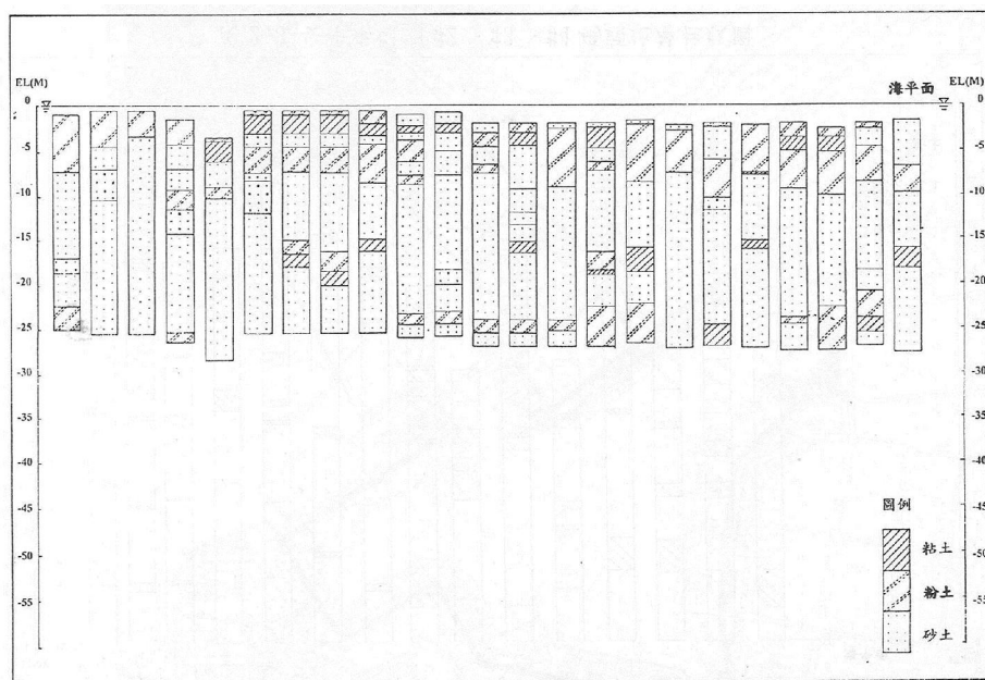
圖 3.4 安平港 5、6、7 號碼頭地層柱狀圖
