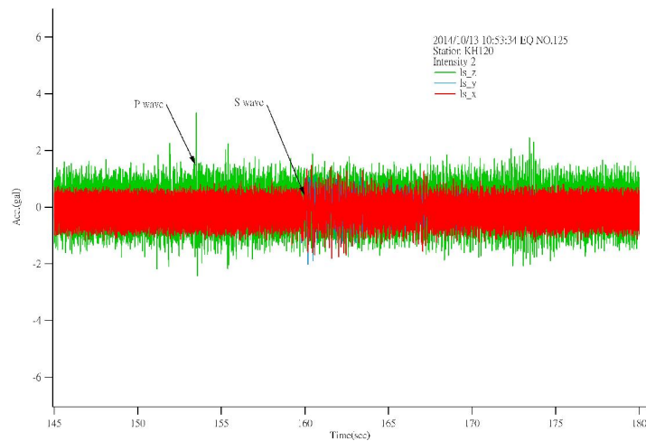
圖 4.13 2014/10/13 KH120 陸上地震儀記錄
