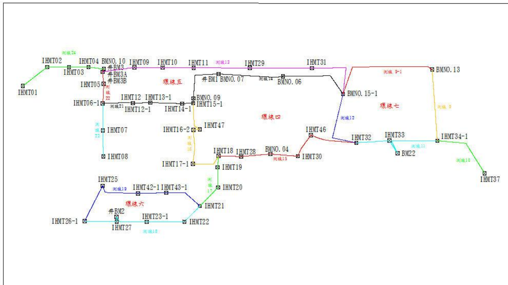
圖 5.14 101 年嘉義縣布袋鎮及布袋港區監測點水準測量水準測線、環線佈置圖
