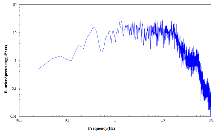
圖 3.13b 安平港 B 類型地震加速度富氏譜圖
