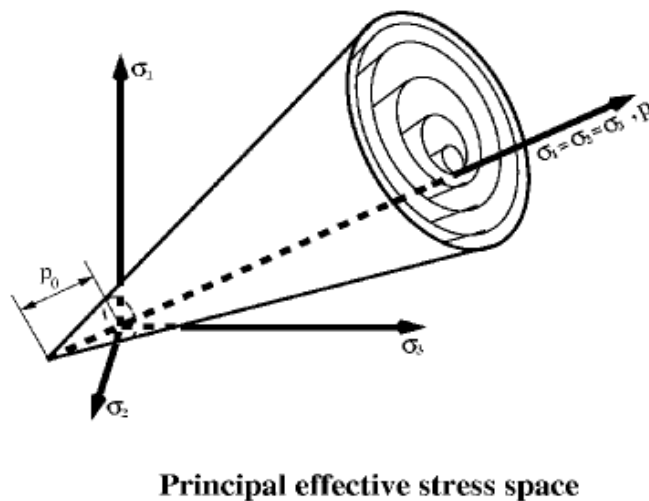
圖 3.24 多重塑性降伏表面空間(Cyclic1D,2004)
