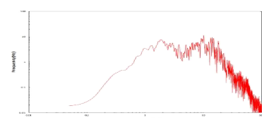
圖 3.13c 安平港 C 類型地震加速度富氏譜圖
