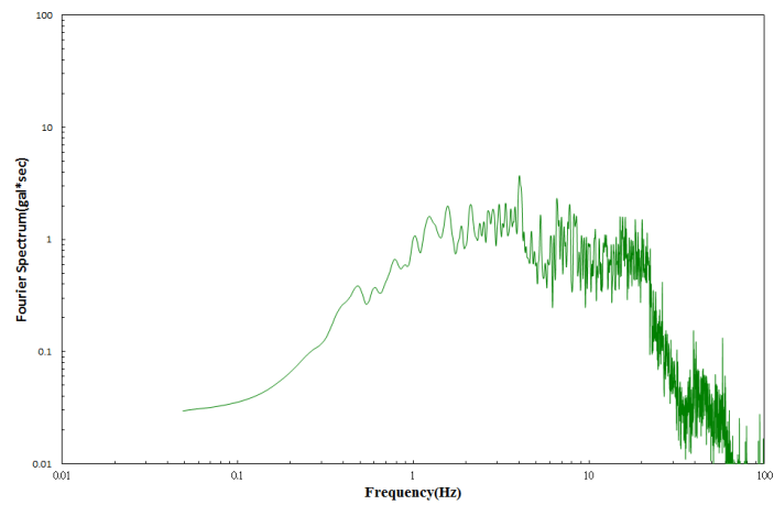
圖 3.13a 安平港 A 類型地震加速度富氏譜圖
