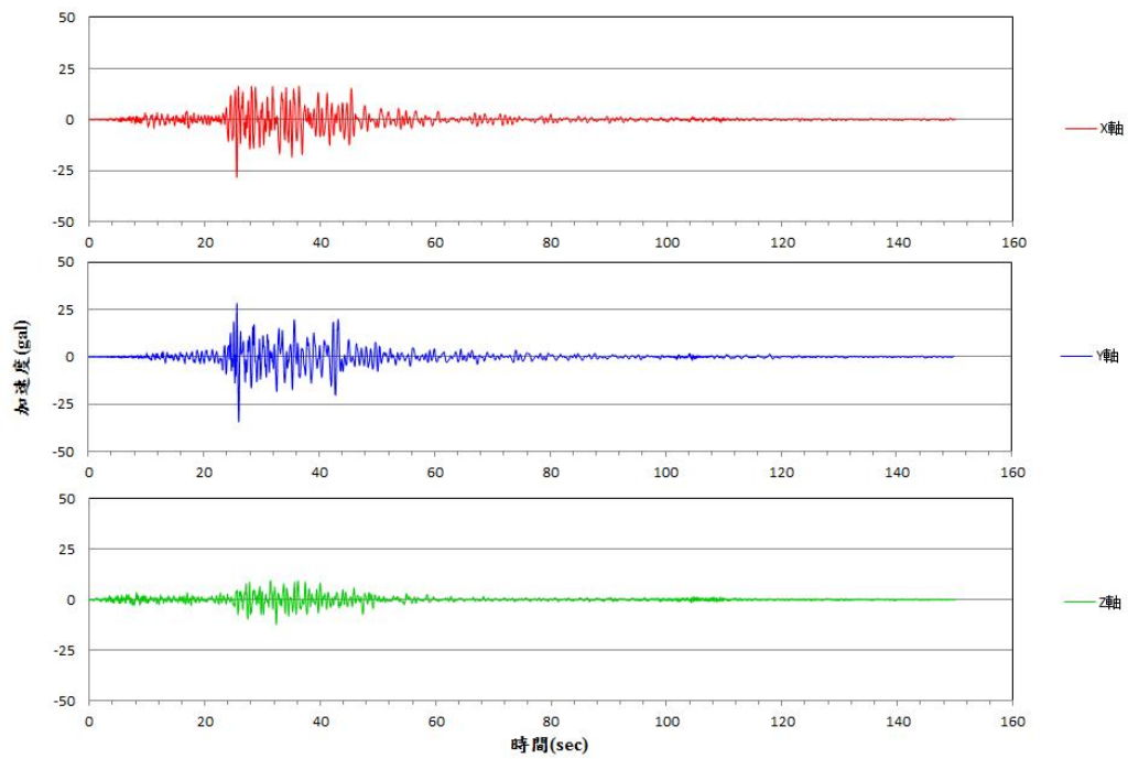
圖 4.22 2013/10/31 臺北港地震站地表加速度計歷時圖
