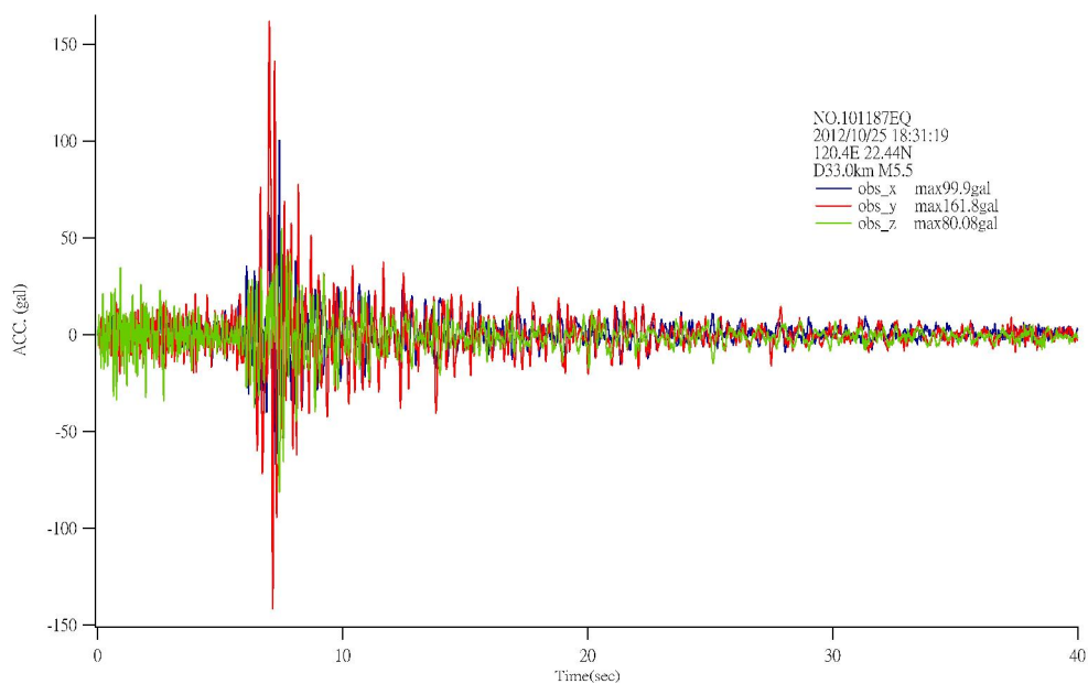
圖 4.9 2012/10/25 KH120 水下地震儀記錄
