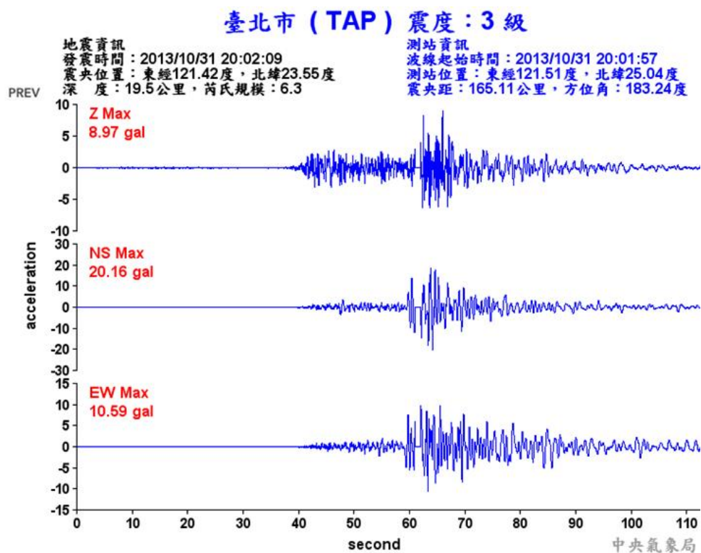
圖 4.20 2013/10/31 臺北市站加速度歷時(氣象局)
