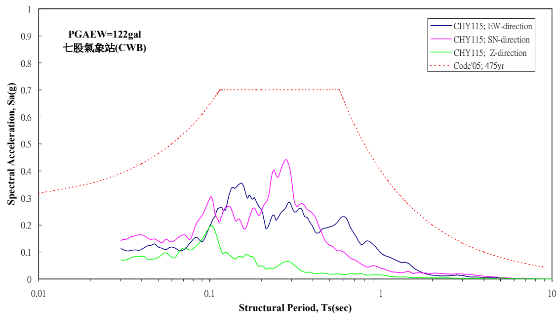
圖 3.46 七股氣象地震站實測反應譜圖(中央氣象局)
