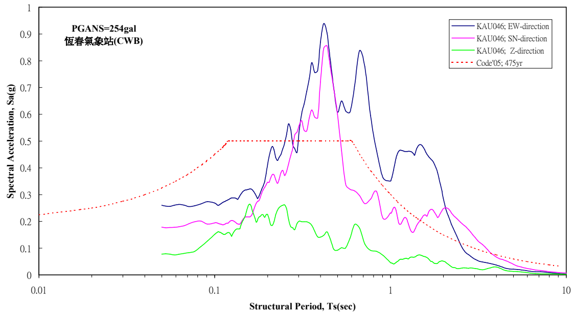
圖 3.44 恆春氣象地震站實測反應譜圖(中央氣象局)
