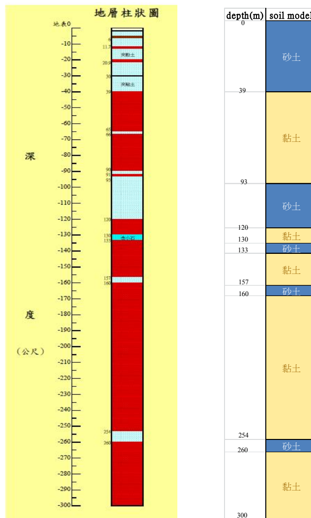
圖 3.26 現地土層柱狀圖與土壤模型對照
