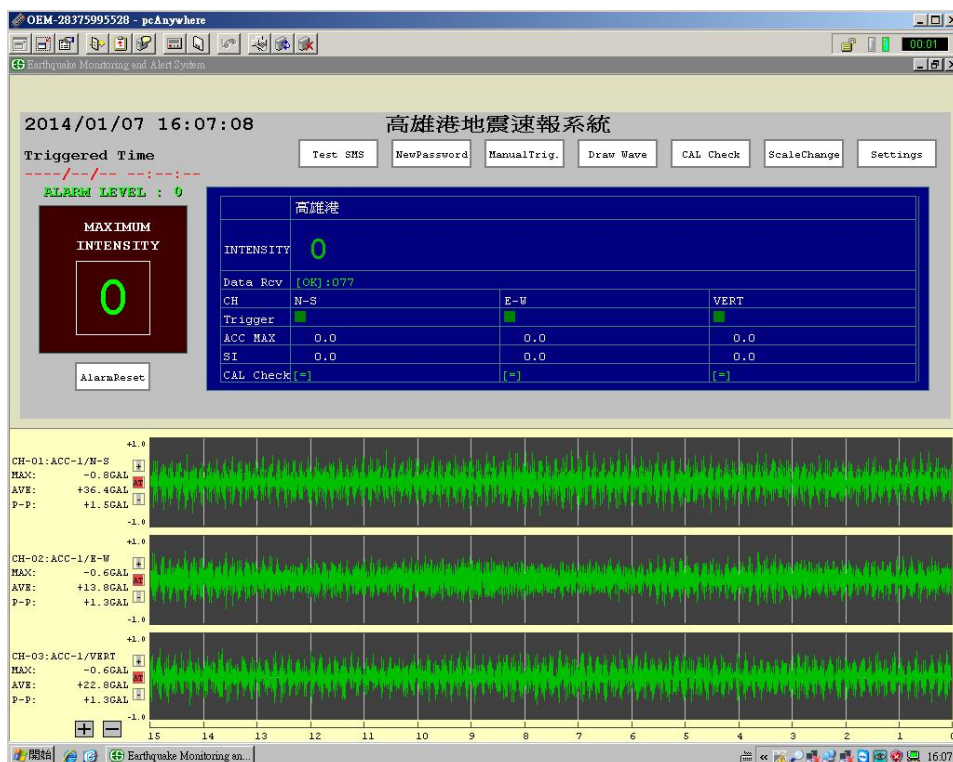
圖 3.40 高雄港區地震即時監測畫面示意圖
