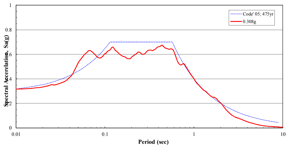
安平港2006~2013年地震水平加速度反應譜平均圖(阻尼比=5%)
