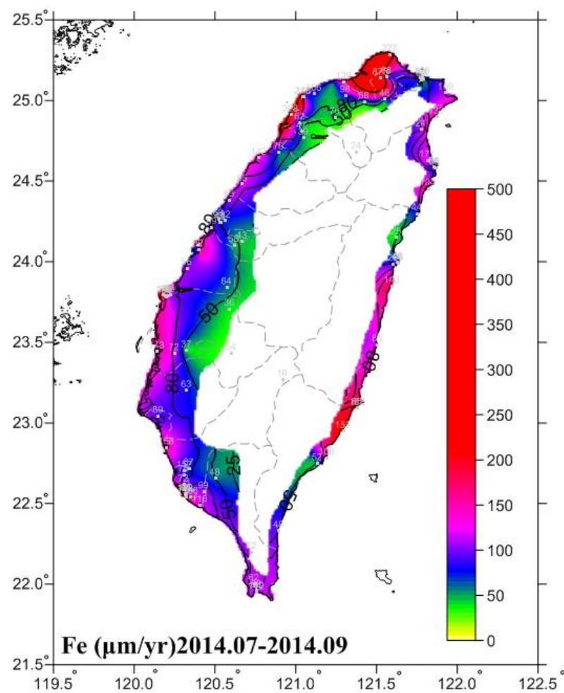
圖 6.11 2014.07-2014.09 碳鋼腐蝕速率圖
