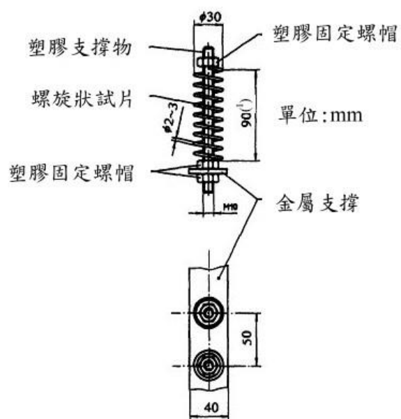
圖 1.4 螺旋狀試片構造示意圖
