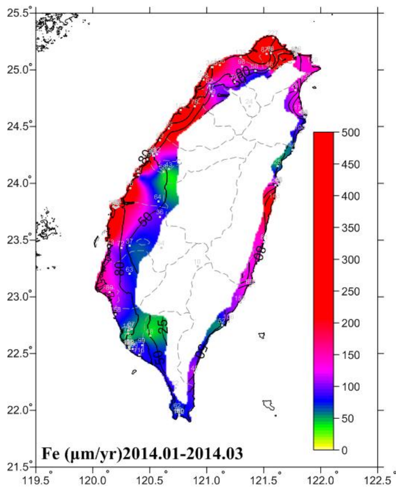
圖 6.9 2014.01-2014.03 碳鋼腐蝕速率圖
