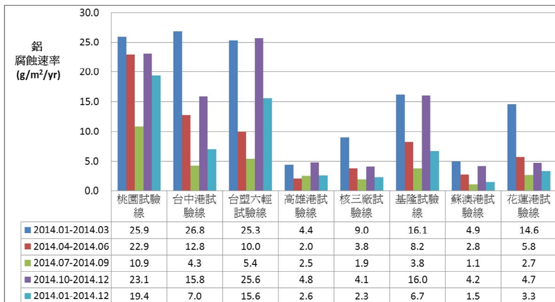
圖 6.4 垂直海岸試驗線鋁腐蝕速率比較圖
