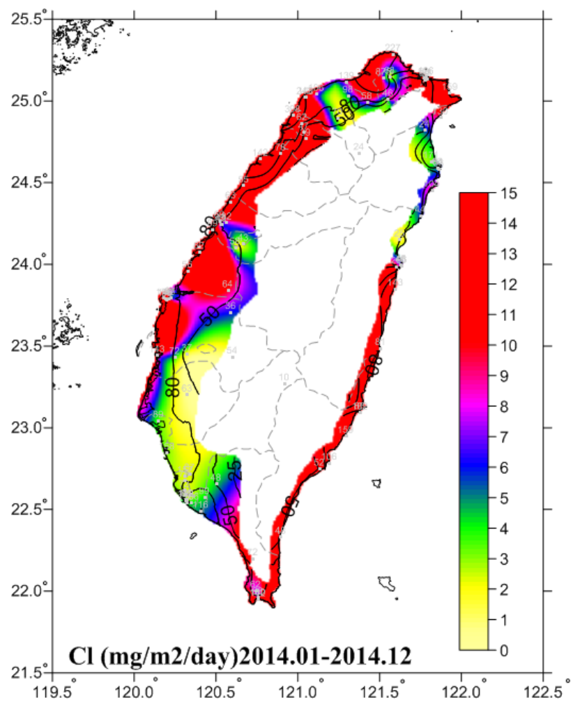
圖 4.5 2014 一年期氯鹽沉積速率圖
