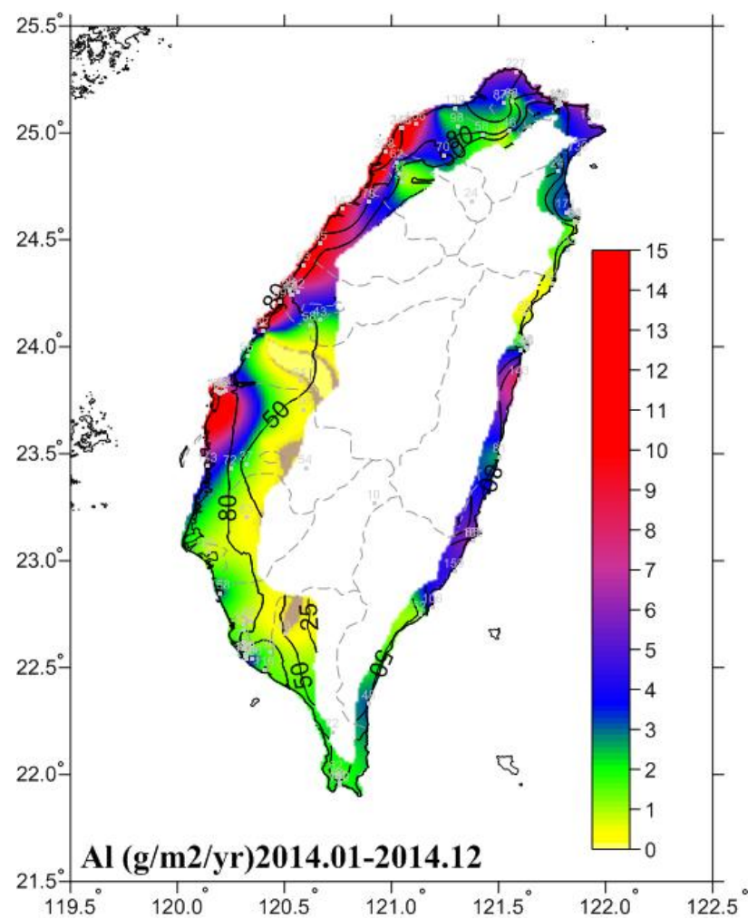
圖 6.28 2014 一年期鋁腐蝕速率
