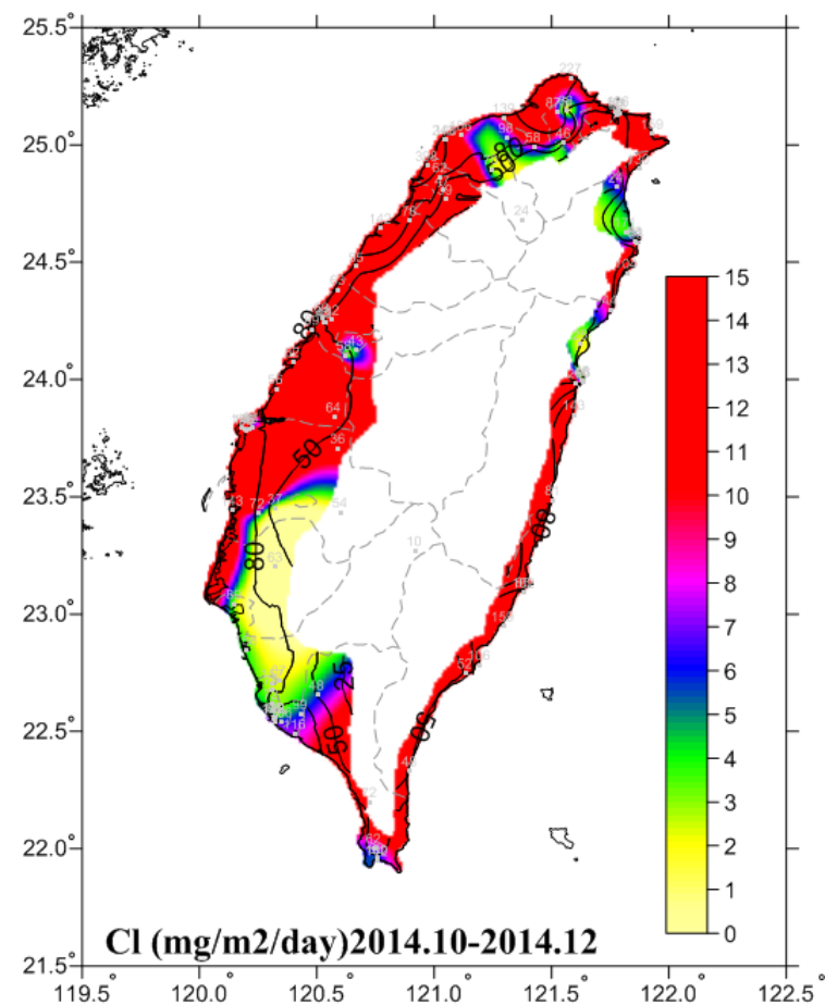
圖 4.4 2014.10-2014.12 氯鹽沉積速率圖
