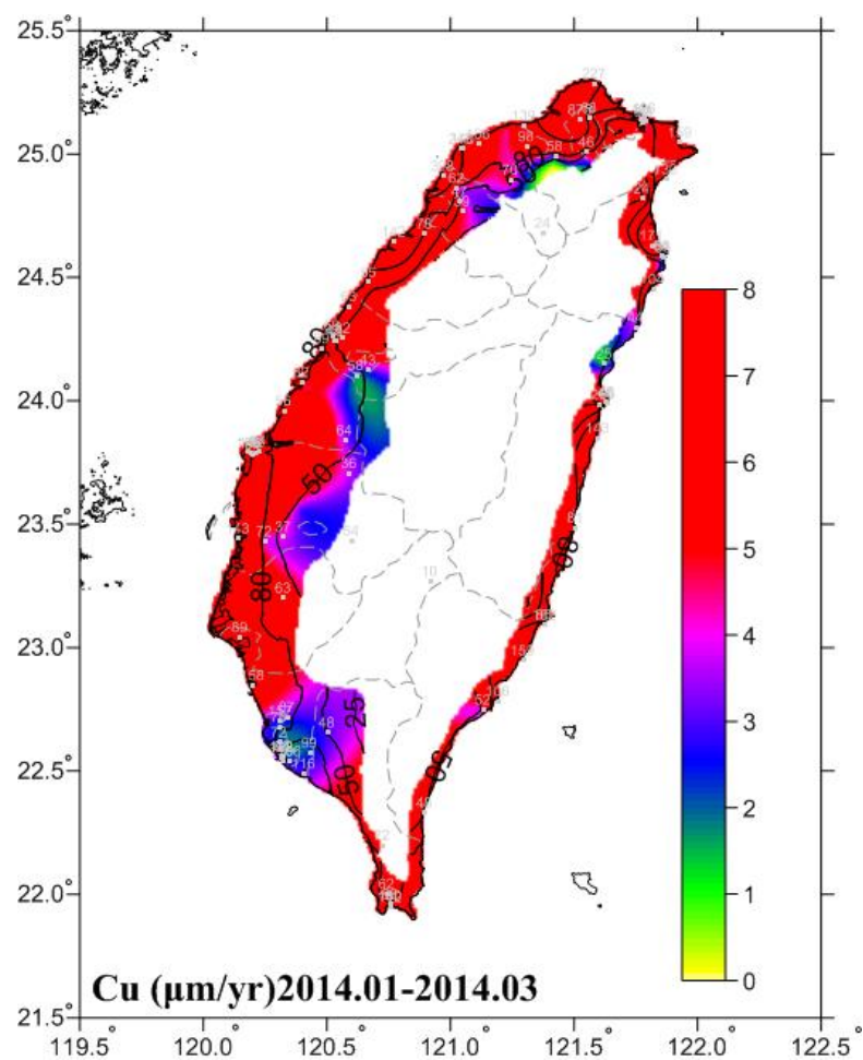
圖 6.17 2014.01-2014.03 銅腐蝕速率圖
