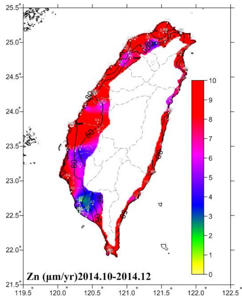
圖 6.16 2014.10-2014.12 鋅腐蝕速率圖
