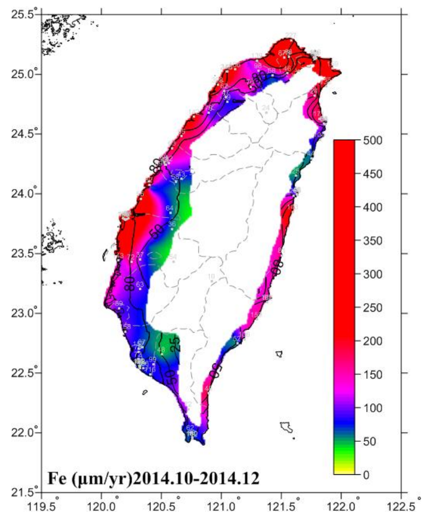
圖 6.12 2014.10-2014.12 碳鋼腐蝕速率圖
