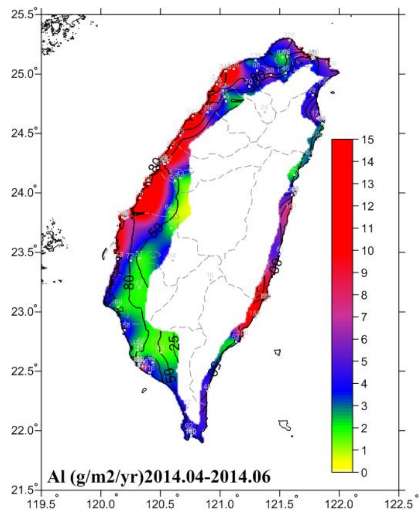
圖 6.22 2014.04-2014.06 鋁腐蝕速率圖
