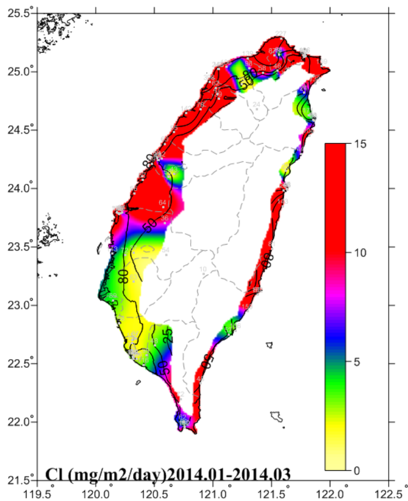
圖 4.1 2014.01-2014.03 氯鹽沉積速率圖
