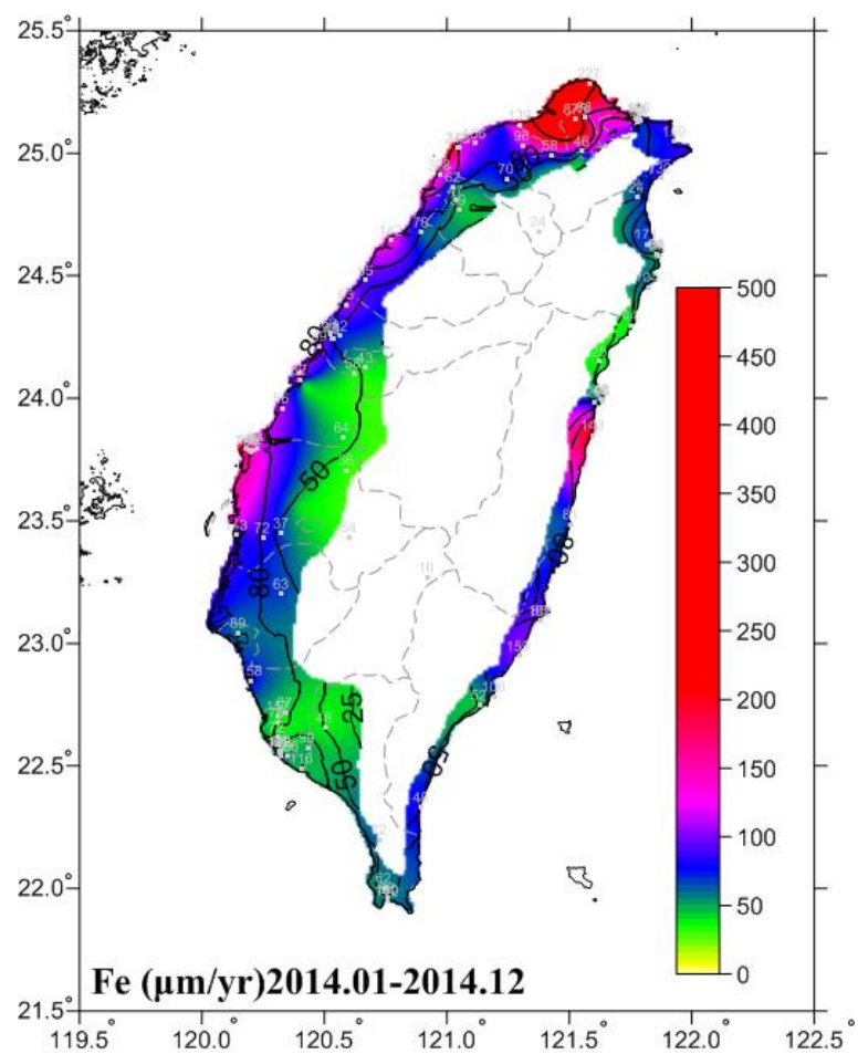
圖 6.25 2014 一年期碳鋼腐蝕速率
