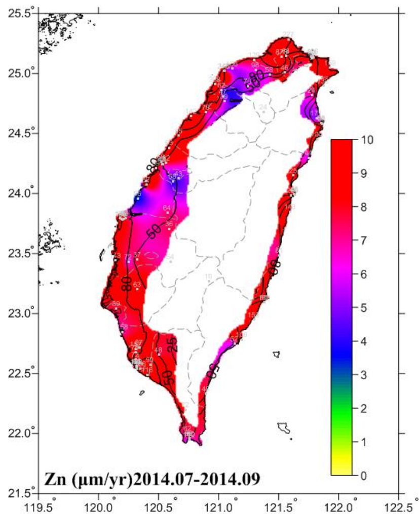
圖 6.15 2014.07-2014.09 鋅腐蝕速率圖
