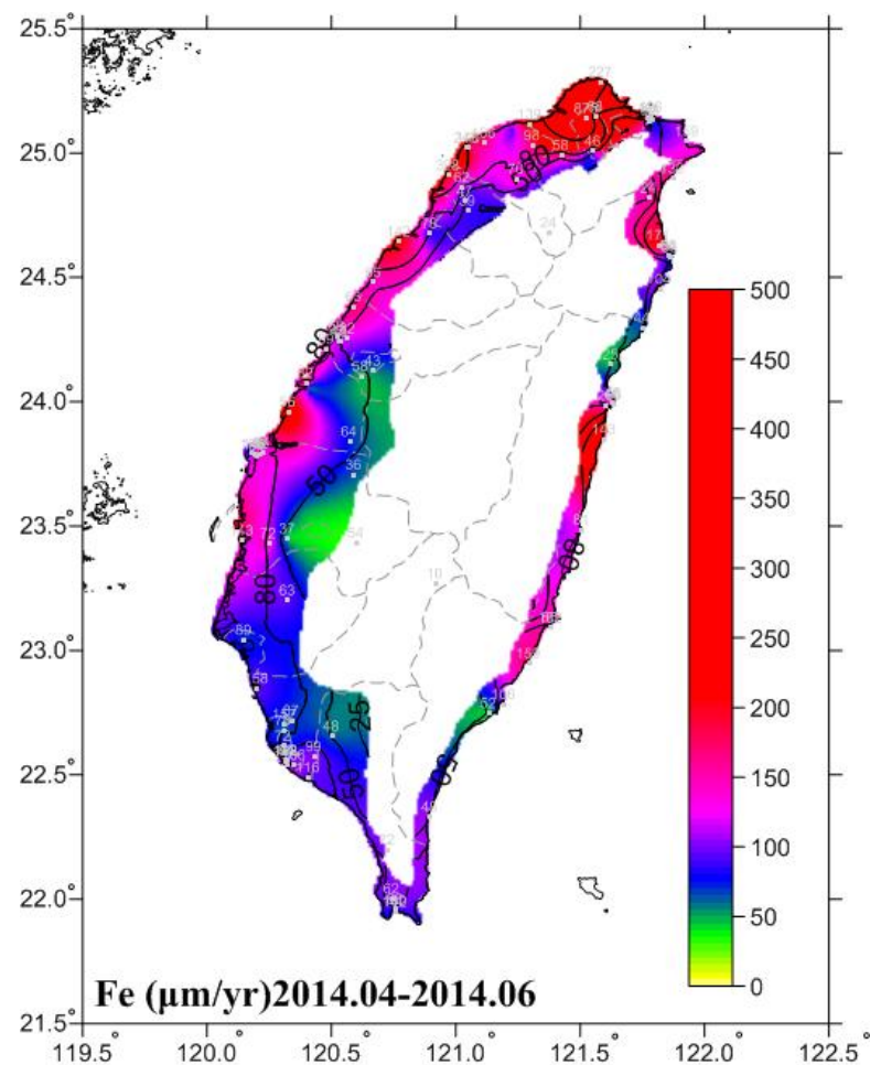
圖 6.10 2014.04-2014.06 碳鋼腐蝕速率圖
