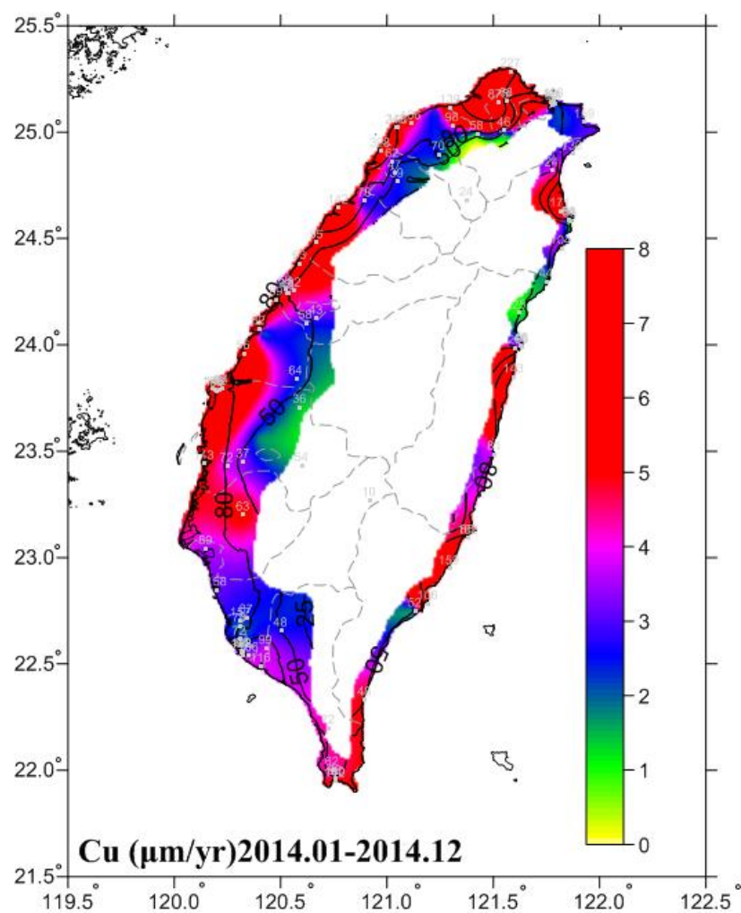
圖 6.27 2014 一年期銅腐蝕速率
