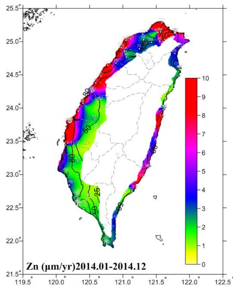
圖 6.26 2014 一年期鋅腐蝕速率
