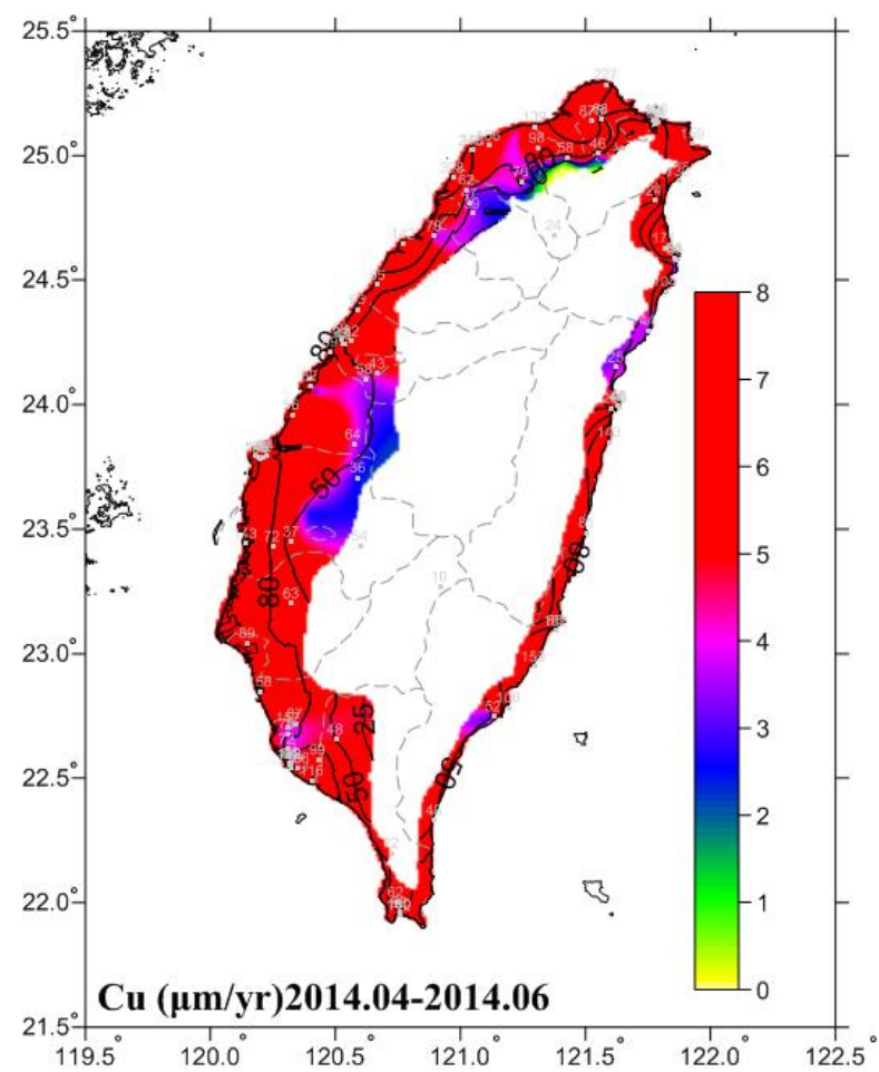
圖 6.18 2014.04-2014.06 銅腐蝕速率圖
