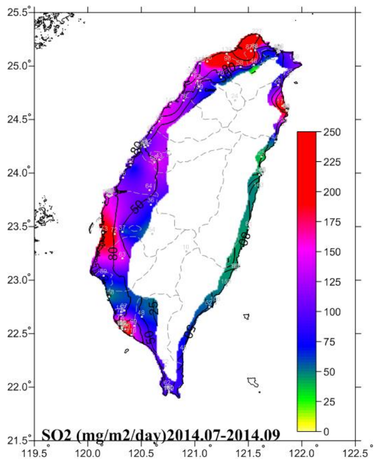
圖 5.3 2014.07-2014.09 二氧化硫沉積速率圖
