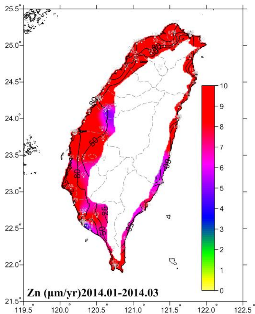
圖 6.13 2014.01-2014.03 鋅腐蝕速率圖
