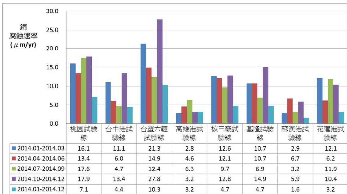
圖 6.3 垂直海岸試驗線銅腐蝕速率比較圖
