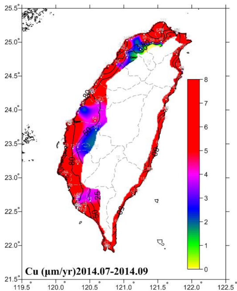
圖 6.19 2014.07-2014.09 銅腐蝕速率圖
