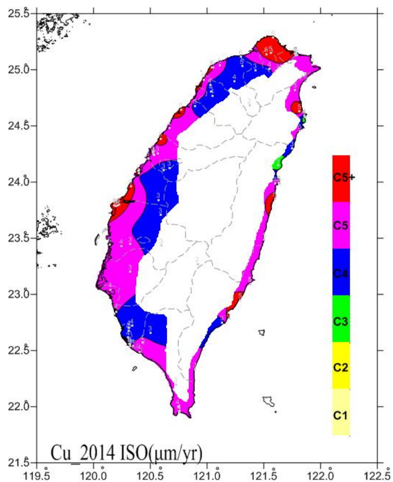
圖 6.31 2014 銅年腐蝕速率 ISO 分類圖
