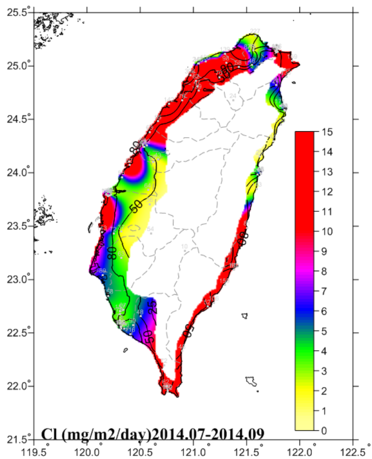
圖 4.3 2014.07-2014.09 氯鹽沉積速率圖
