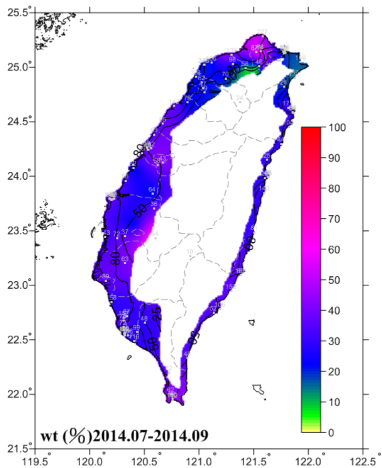
圖 3.3 2014.07-2014.09 濕潤時間圖
