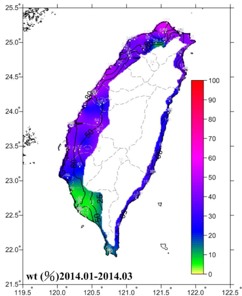
圖 3.1 2014.01-2014.03 濕潤時間圖
