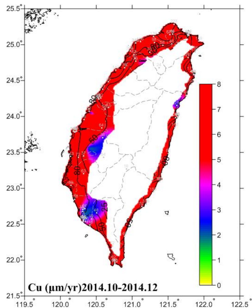
圖 6.20 2014.10-2014.12 銅腐蝕速率圖
