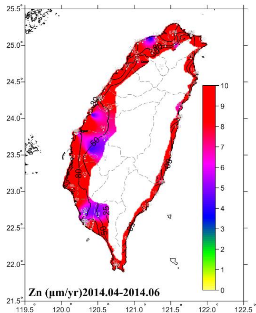
圖 6.14 2014.04-2014.06 鋅腐蝕速率圖
