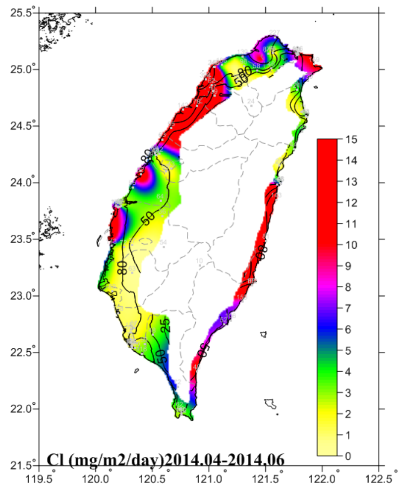
圖 4.2 2014.04-2014.06 氯鹽沉積速率圖
