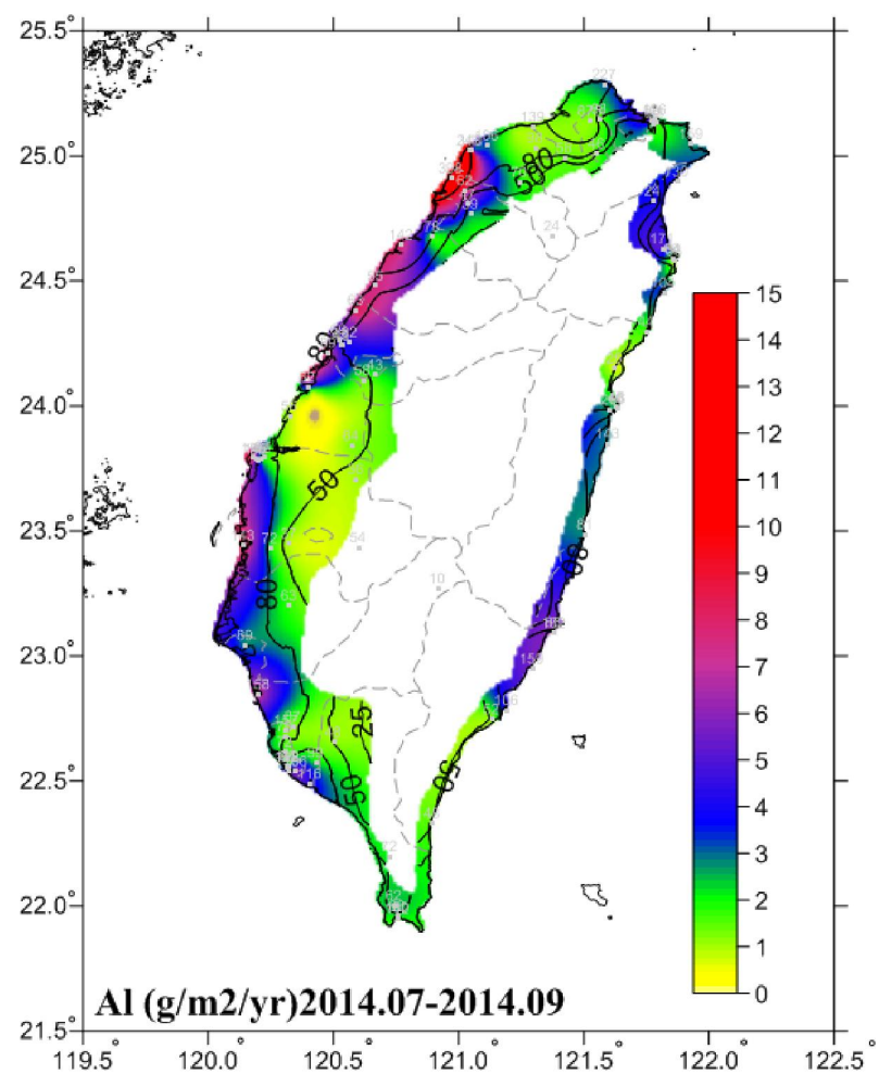
圖 6.23 2014.07-2014.09 鋁腐蝕速率圖
