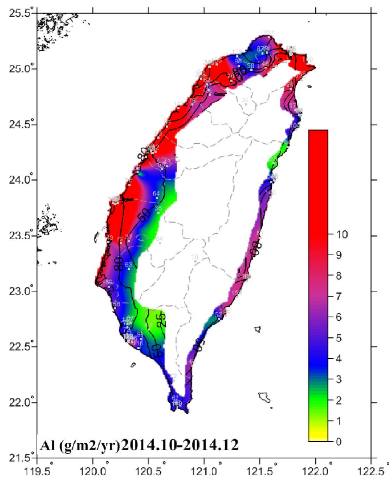
圖 6.24 2014.10-2014.12 鋁腐蝕速率圖
