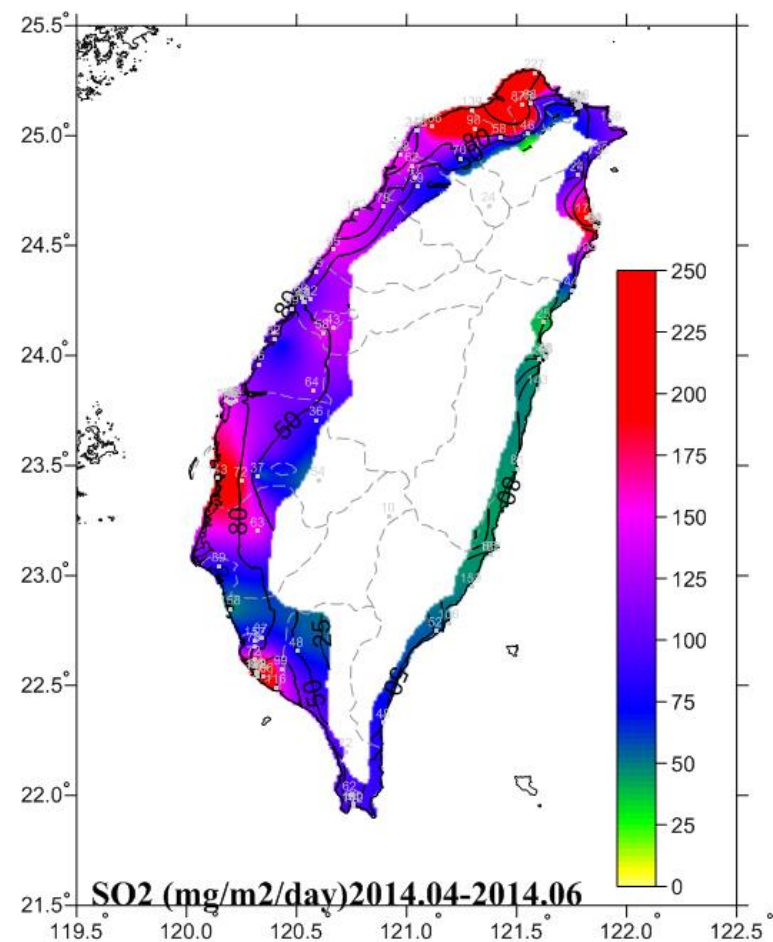
圖 5.2 2014.04-2014.06 二氧化硫沉積速率圖
