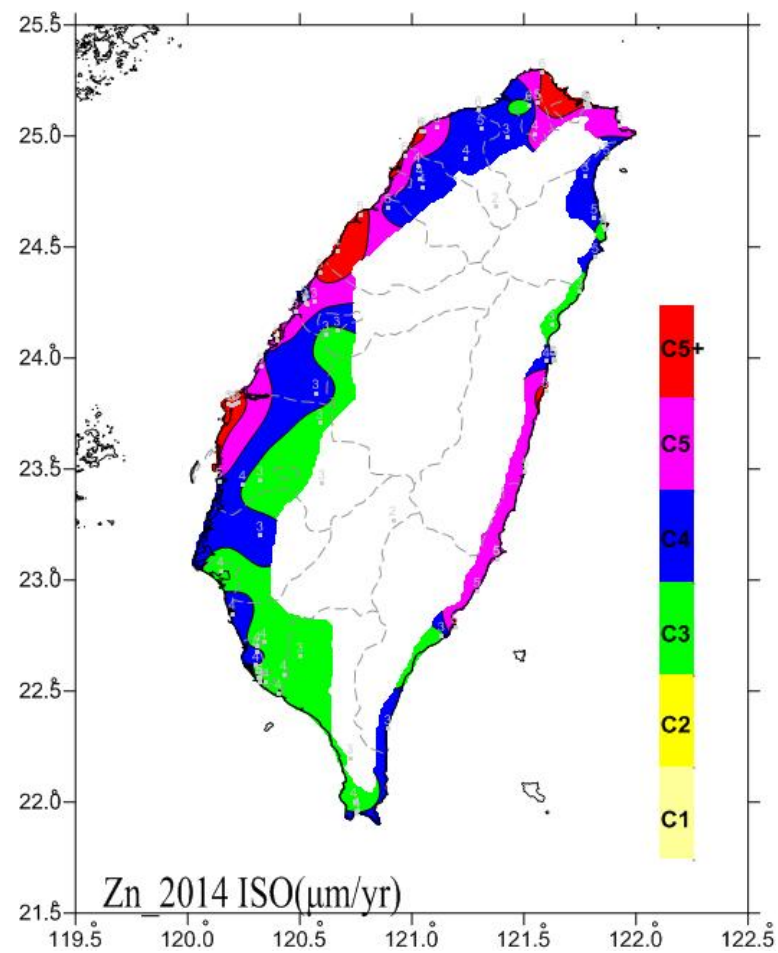
圖 6.30 2014 鋅年腐蝕速率 ISO 分類圖
