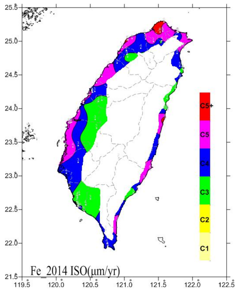
圖 6.29 2014 碳鋼年腐蝕速率 ISO 分類圖
