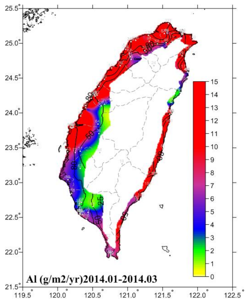
圖 6.21 2014.01-2014.03 鋁腐蝕速率圖
