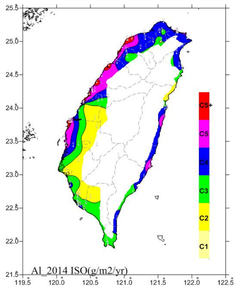
圖 6.32 2014 鋁年腐蝕速率 ISO 分類圖
