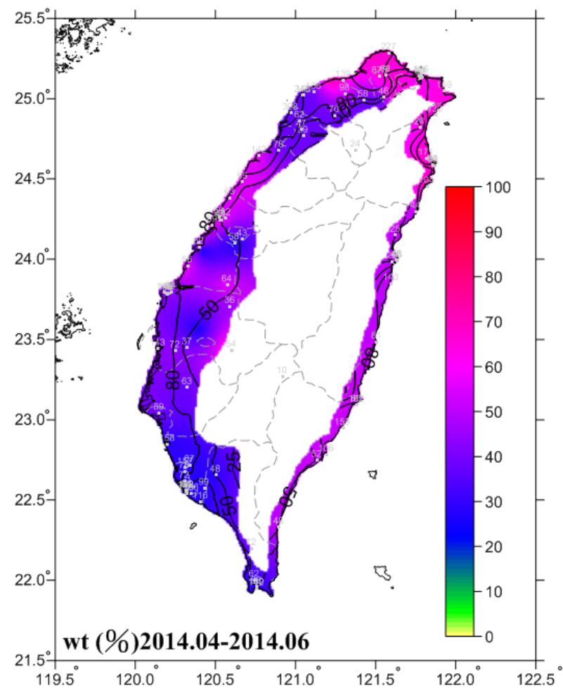
圖 3.2 2014.04-2014.06 濕潤時間圖
