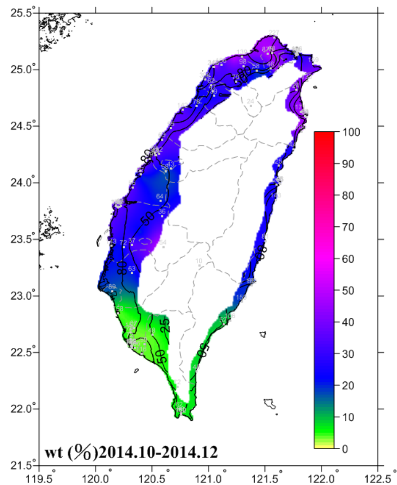
圖 3.4 2014.10-2014.12 濕潤時間圖
