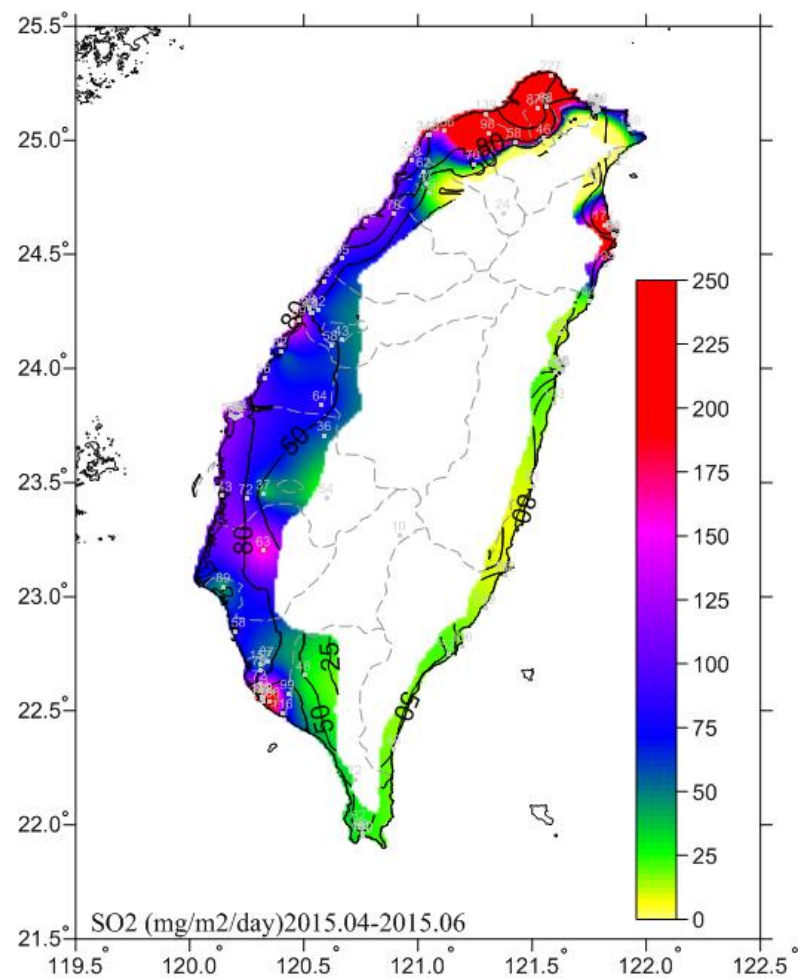
圖 5.2 2015.04-2015.06 二氧化硫沉積速率圖
