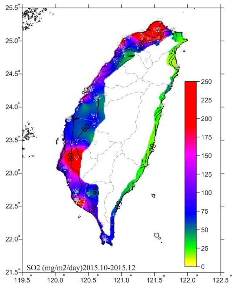
圖 5.4 2015.10-2015.12 二氧化硫沉積速率圖
