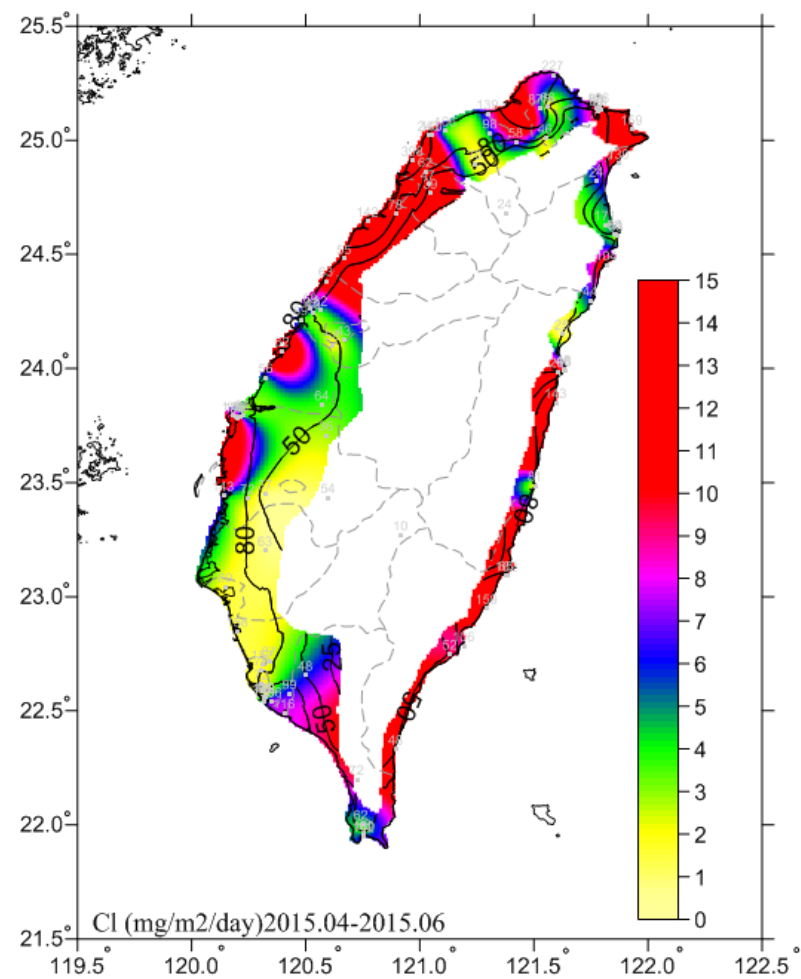
圖 4.2 2015.04-2015.06 氯鹽沉積速率圖
