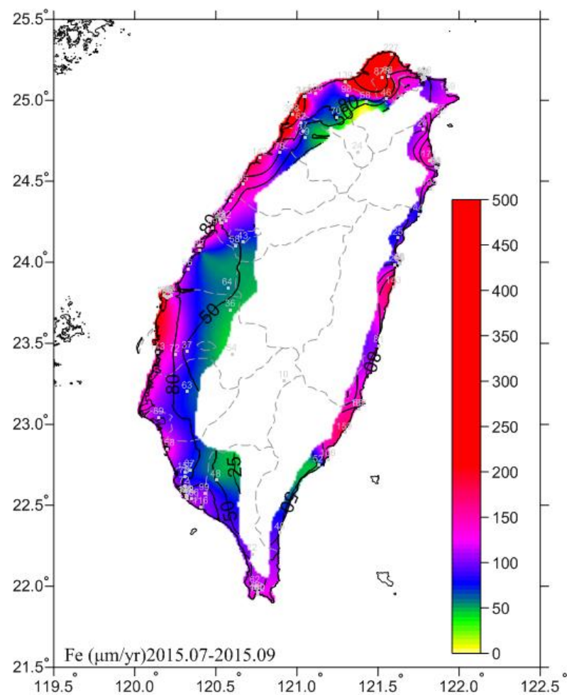
圖 6.11 2015.07-2015.09 碳鋼腐蝕速率圖
