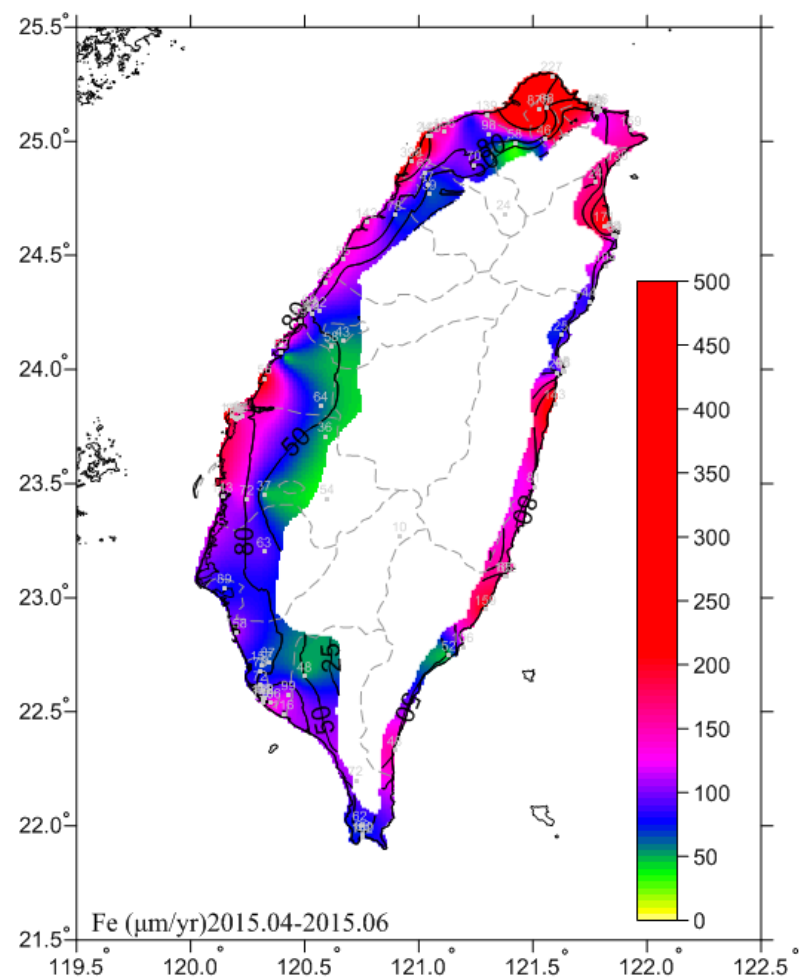
圖 6.10 2015.04-2015.06 碳鋼腐蝕速率圖
