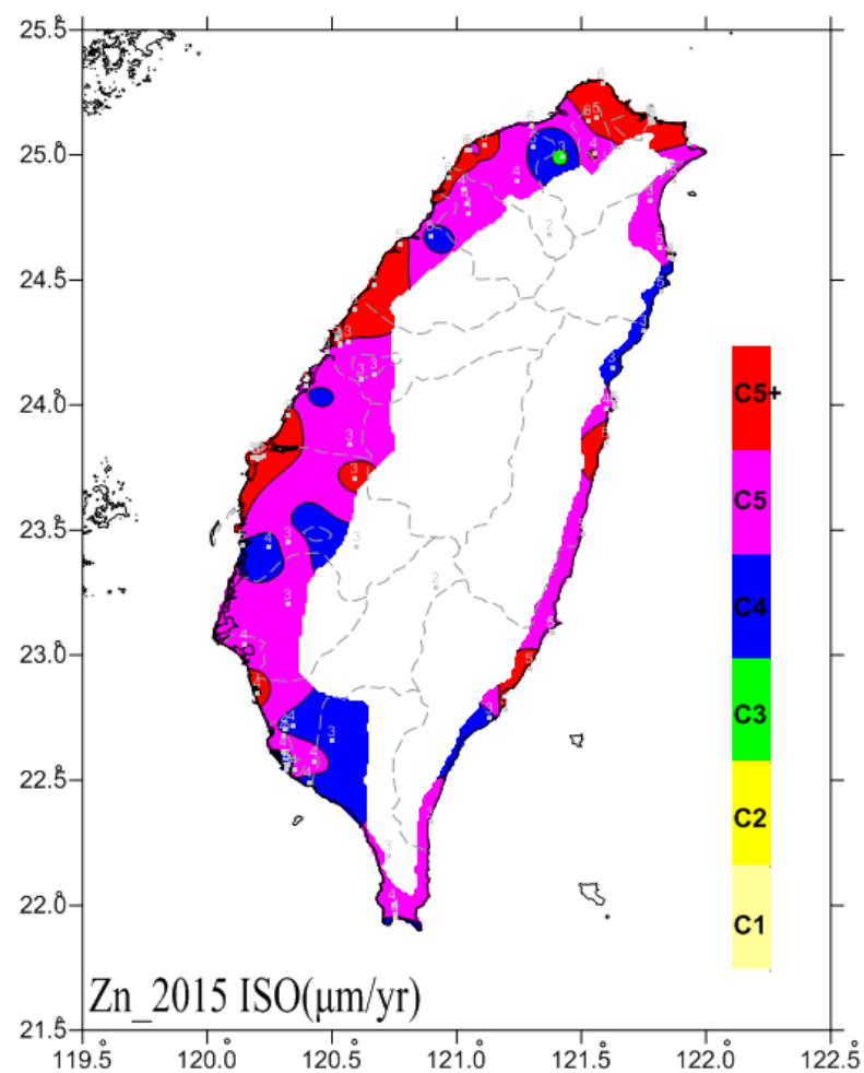
圖 6.30 2015 鋅年腐蝕速率 ISO 分類圖
