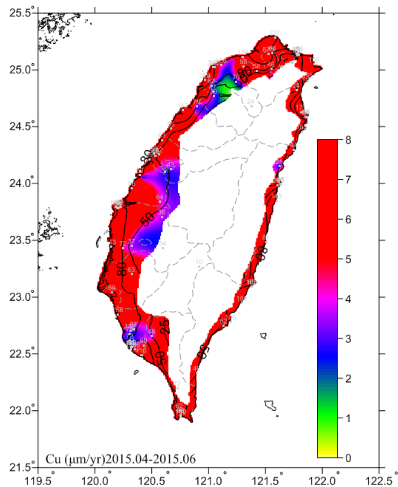
圖 6.18 2015.04-2015.06 銅腐蝕速率圖
