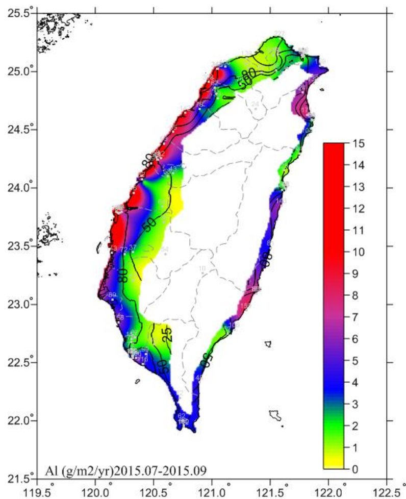
圖 6.23 2015.07-2015.09 鋁腐蝕速率圖
