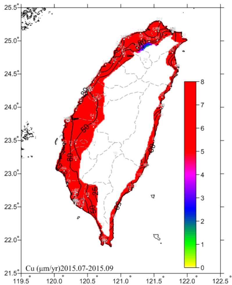
圖 6.19 2015.07-2015.09 銅腐蝕速率圖
