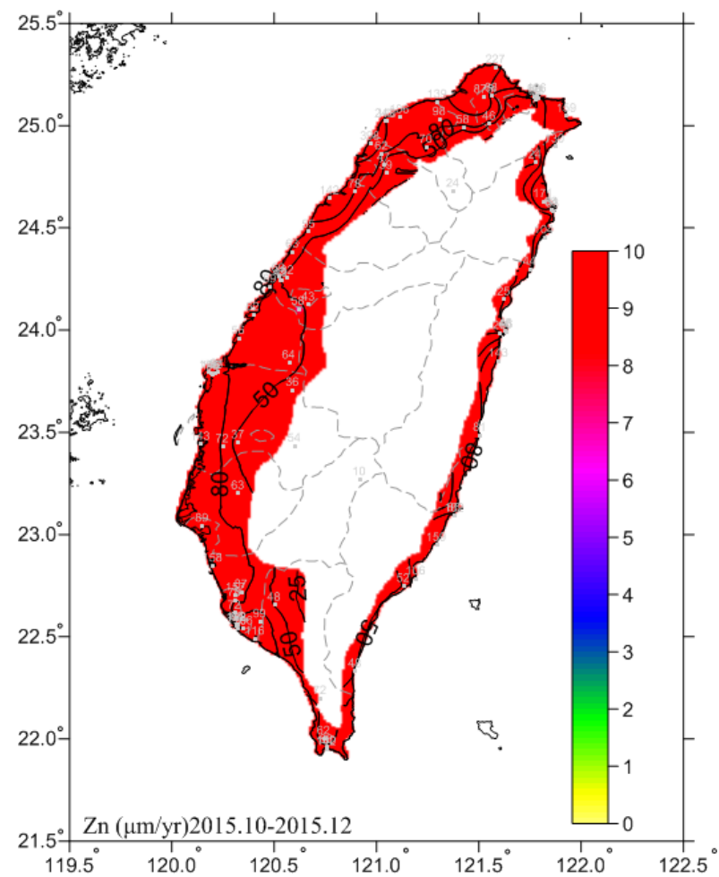
圖 6.16 2015.10-2015.12 鋅腐蝕速率圖
