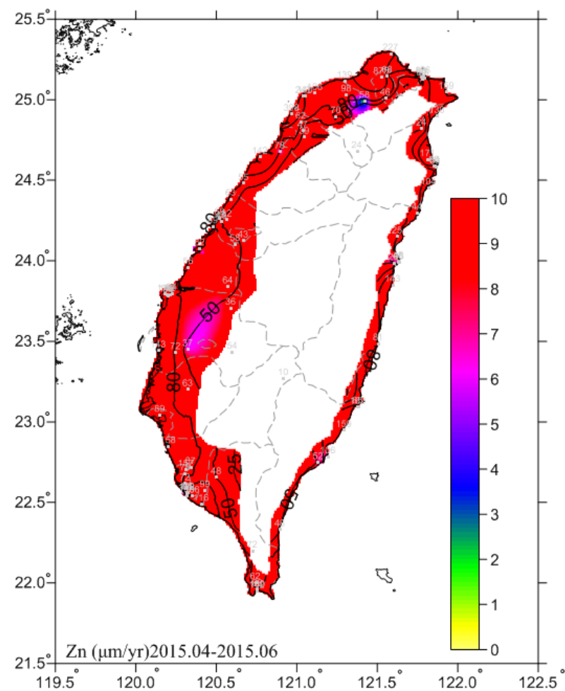
圖 6.14 2015.04-2015.06 鋅腐蝕速率圖
