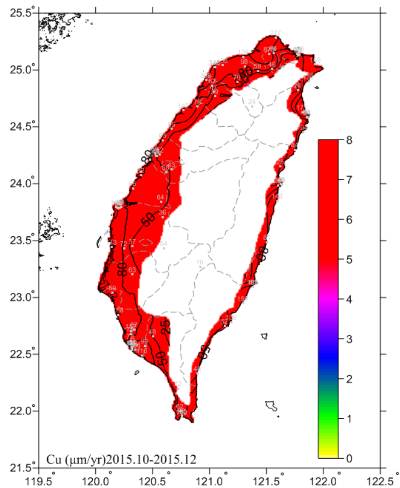
圖 6.20 2015.10-2015.12 銅腐蝕速率圖
