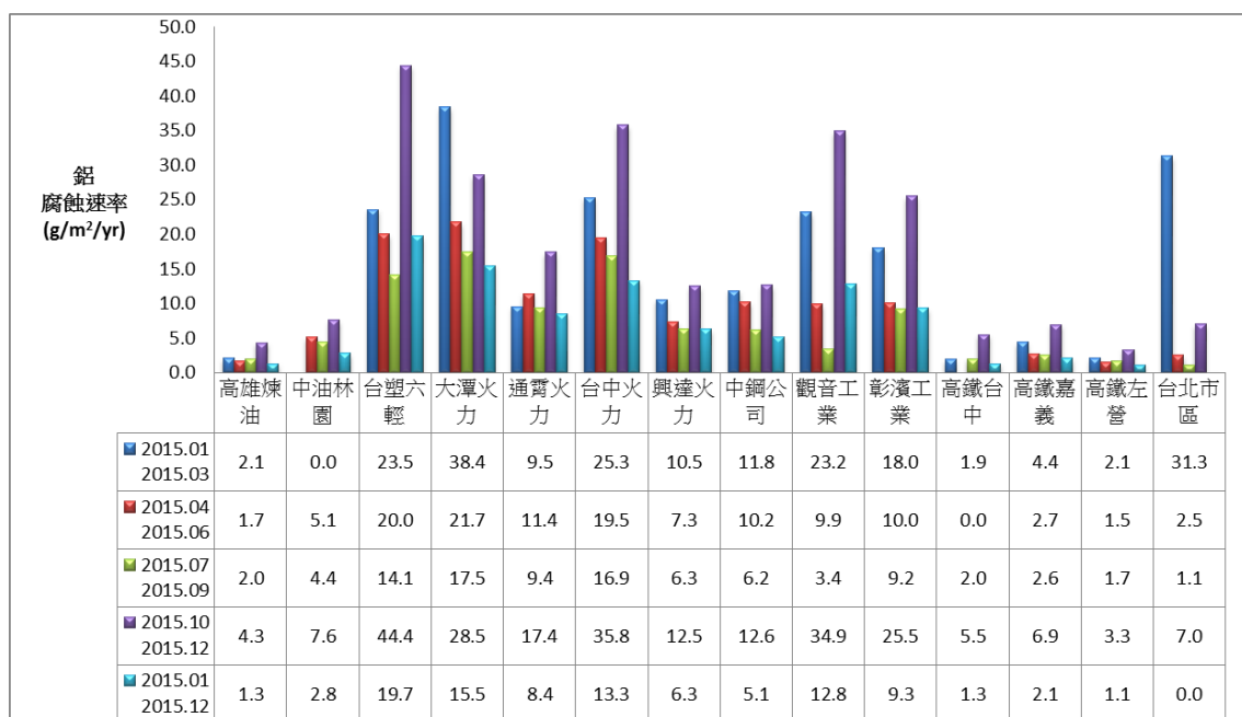
圖 6.7 特定測站銅腐蝕速率比較圖
