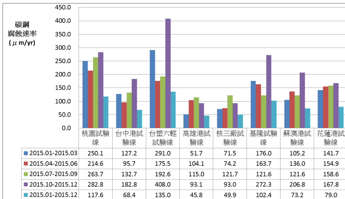
圖 6.1 垂直海岸試驗線碳鋼腐蝕速率比較圖
