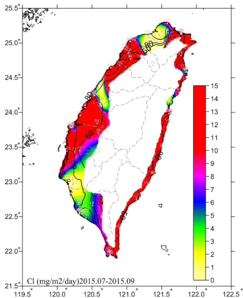
圖 4.3 2015.07-2015.09 氯鹽沉積速率圖
