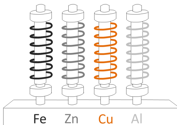
圖 1.5 金屬線材試樣暴露裝置圖
