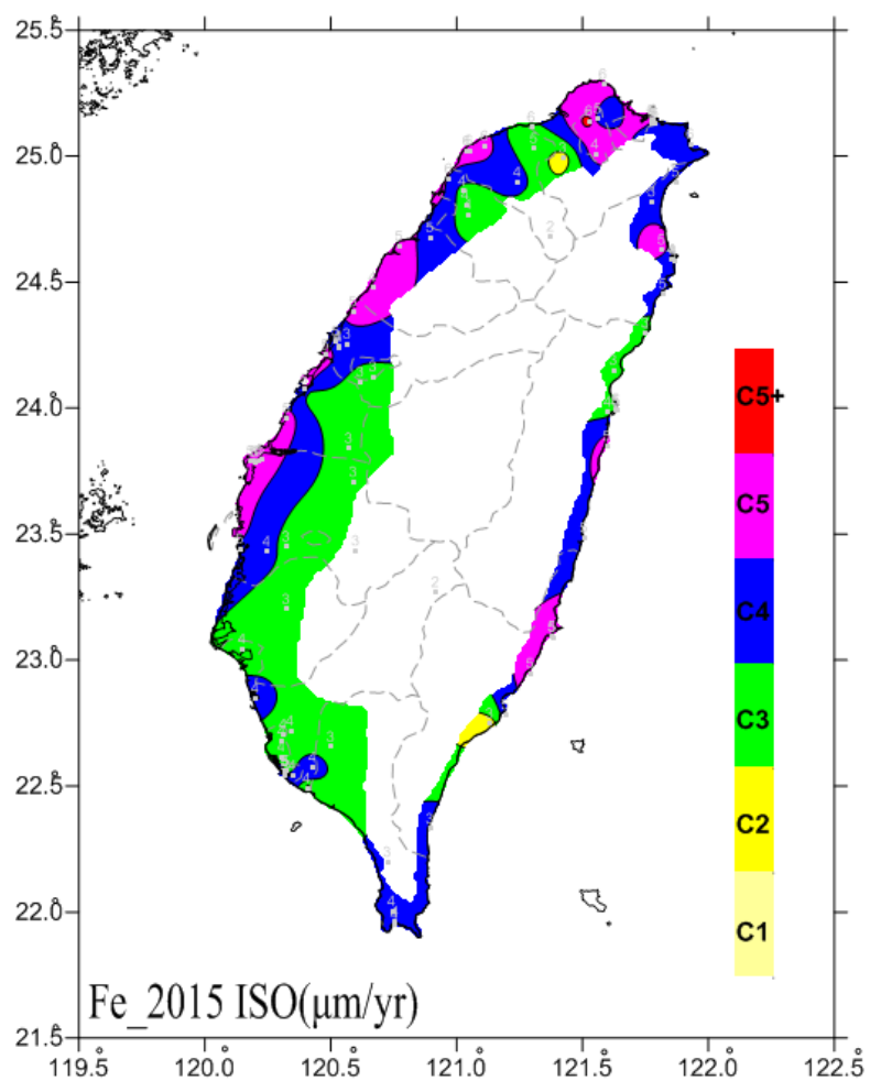
圖 6.29 2015 碳鋼年腐蝕速率 ISO 分類圖
