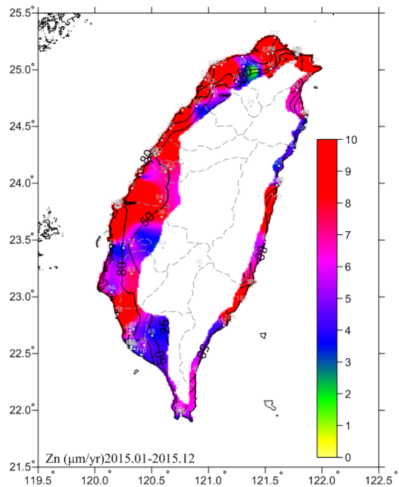
圖 6.26 2015 一年期鋅腐蝕速率
