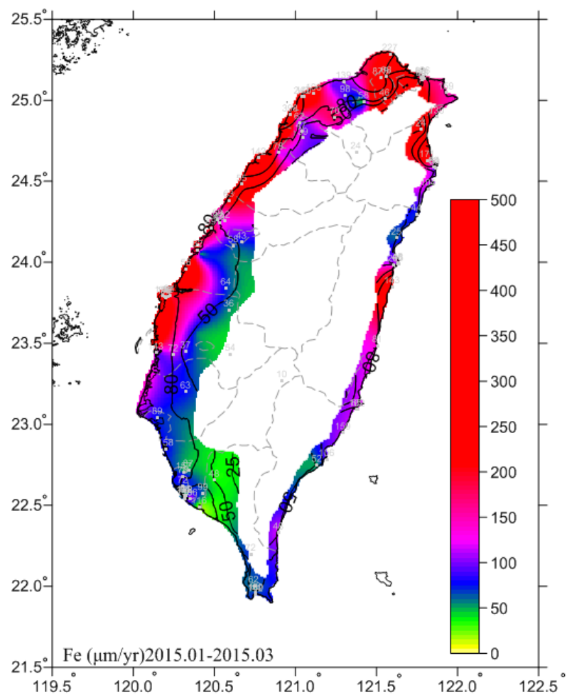
圖 6.9 2015.01-2015.03 碳鋼腐蝕速率圖
