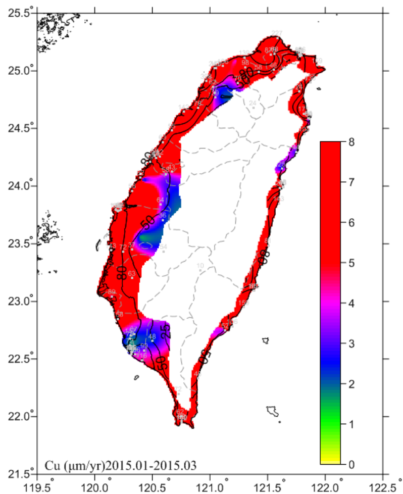
圖 6.17 2015.01-2015.03 銅腐蝕速率圖
