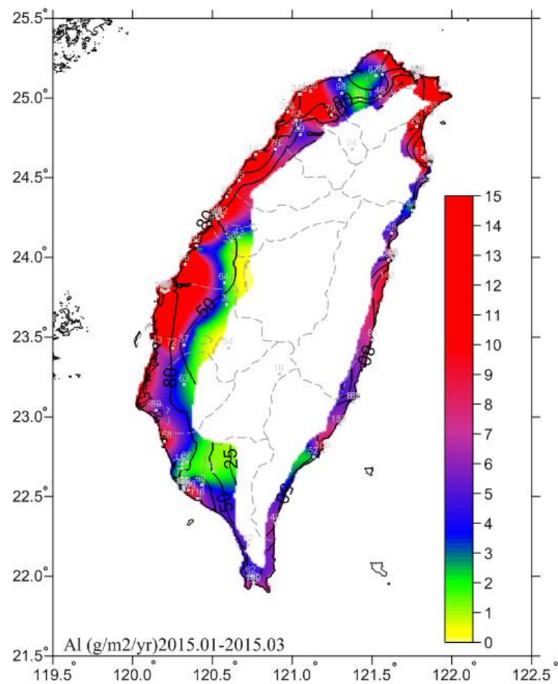
圖 6.21 2015.01-2015.03 鋁腐蝕速率圖
