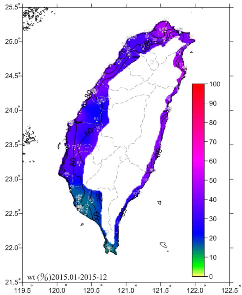
圖 3.5 2015 一年期濕潤時間圖
