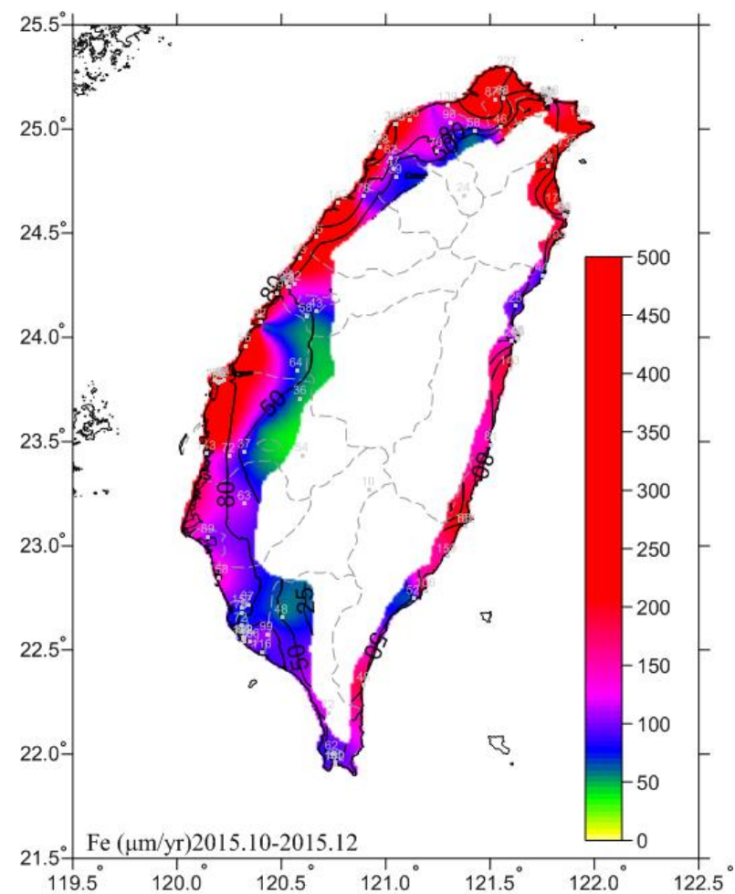
圖 6.12 2015.10-2015.12 碳鋼腐蝕速率圖
