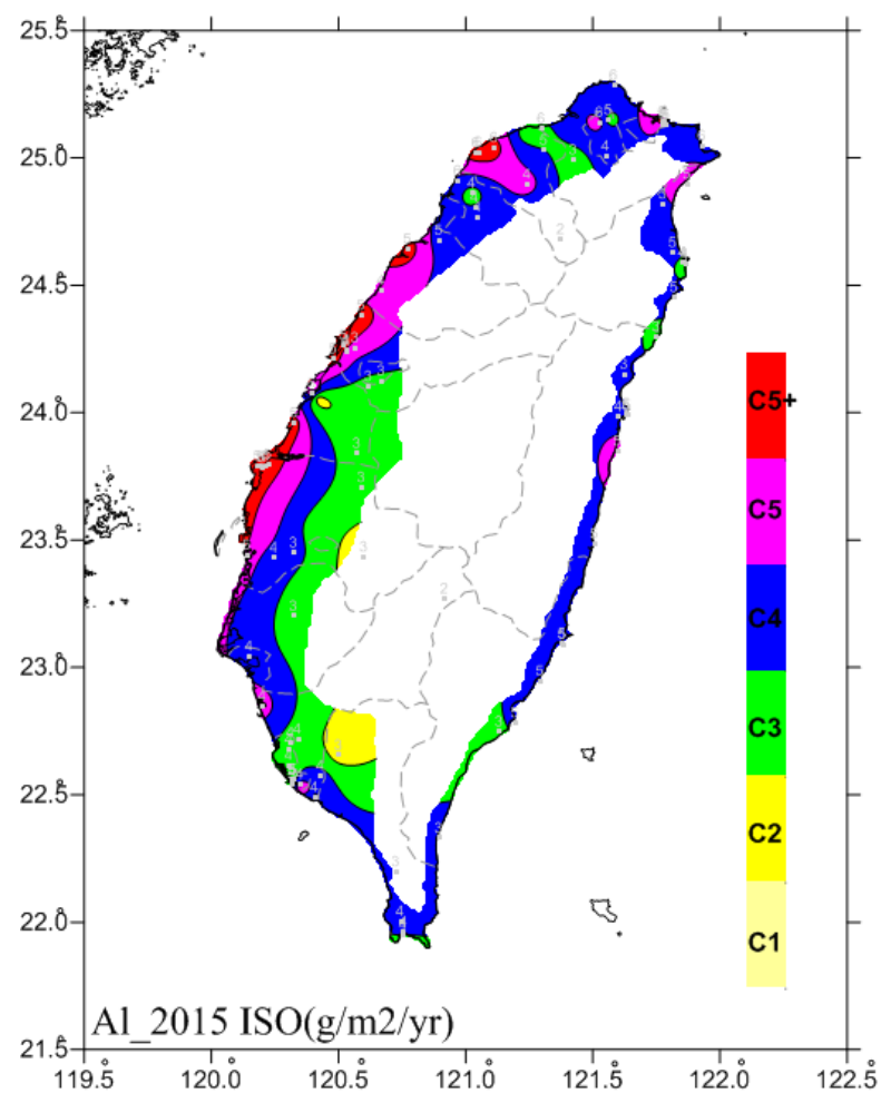
圖 6.32 2015 鋁年腐蝕速率 ISO 分類圖
