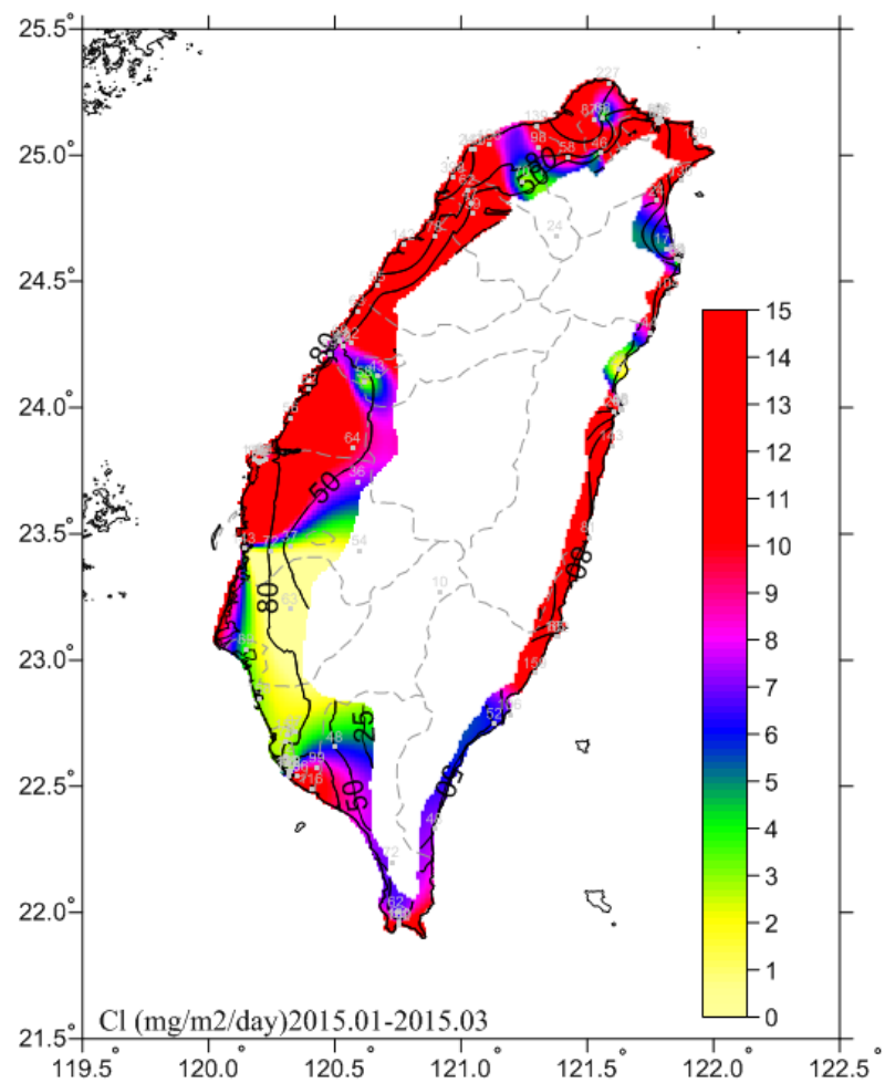
圖 4.1 2015.01-2015.03 氯鹽沉積速率圖
