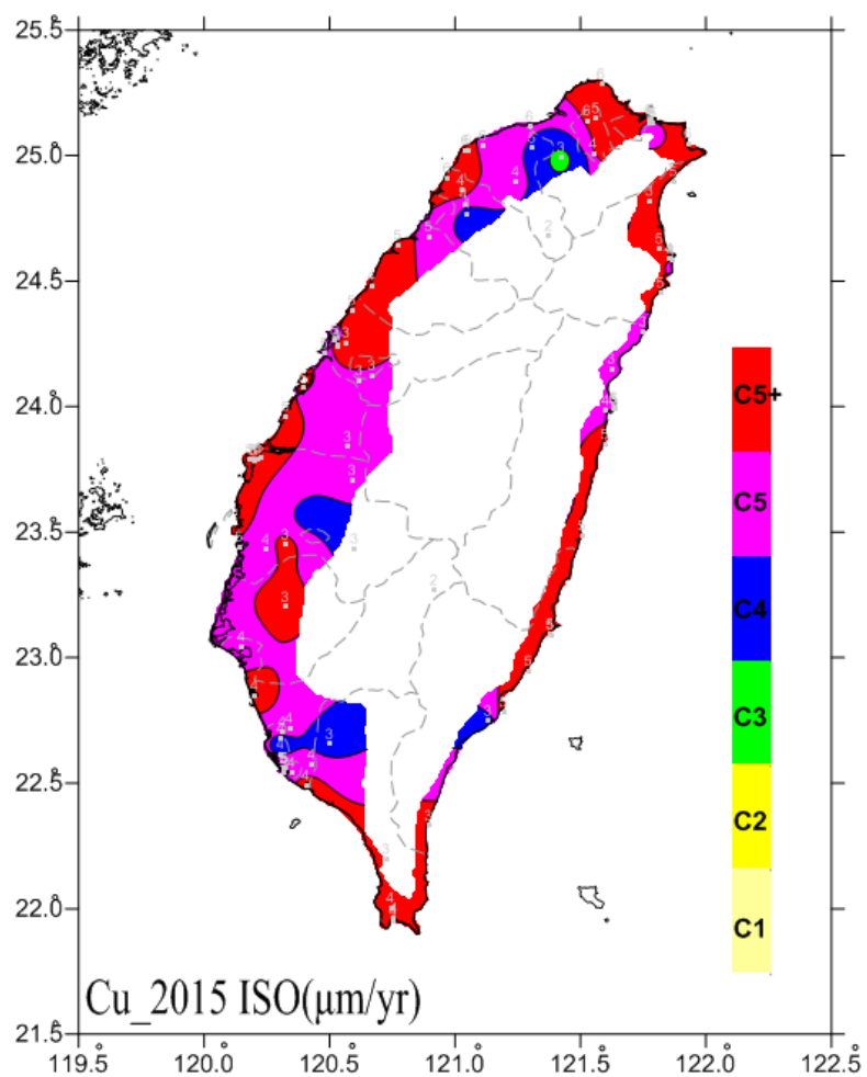
圖 6.31 2015 銅年腐蝕速率 ISO 分類圖
