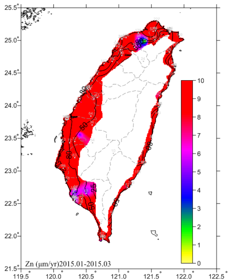
圖 6.13 2015.01-2015.03 鋅腐蝕速率圖
