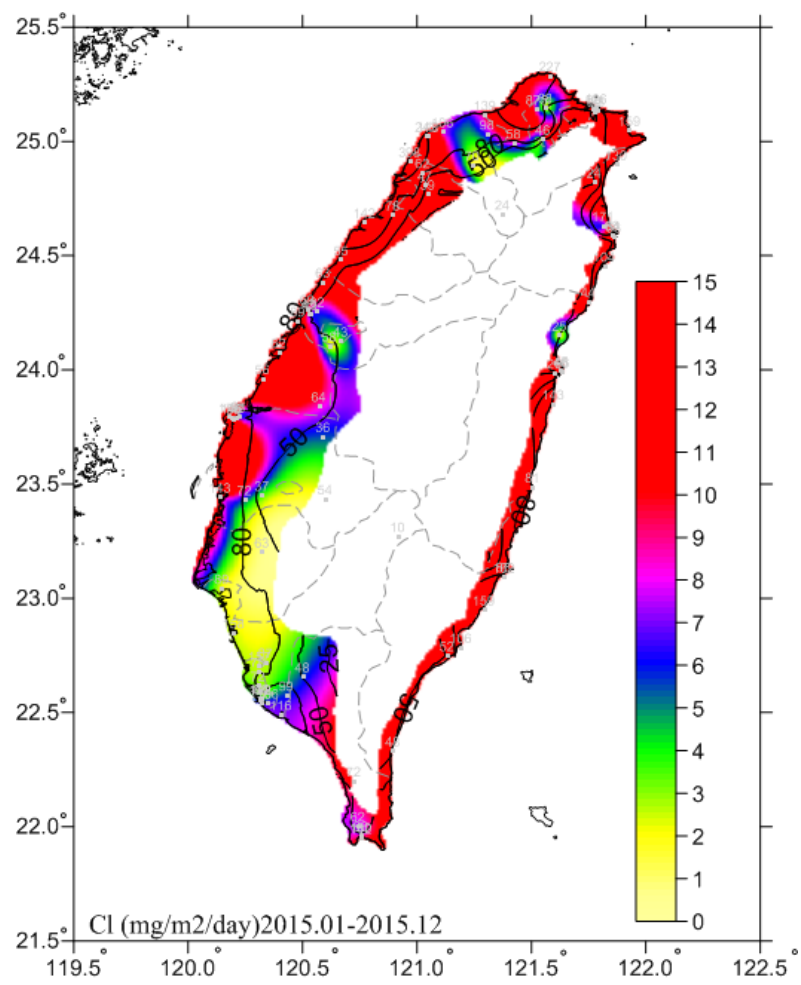
圖 4.5 2015 一年期氯鹽沉積速率圖
