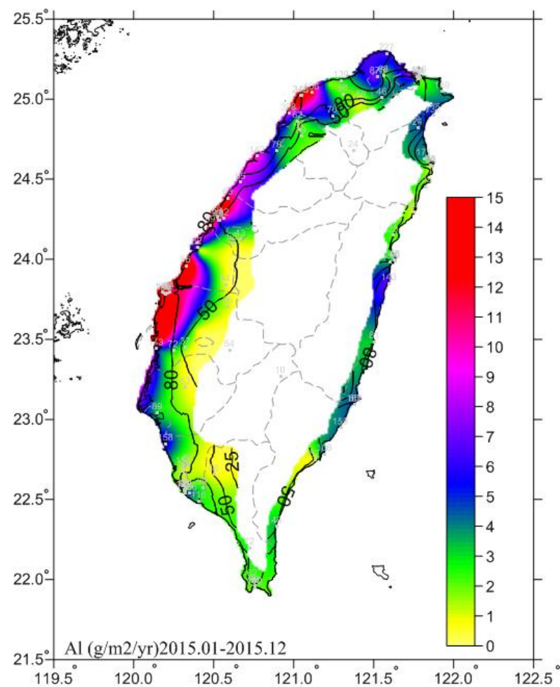
圖 6.28 2015 一年期鋁腐蝕速率
