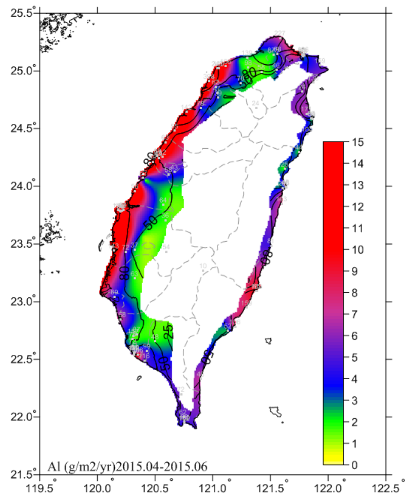
圖 6.22 2015.04-2015.06 鋁腐蝕速率圖
