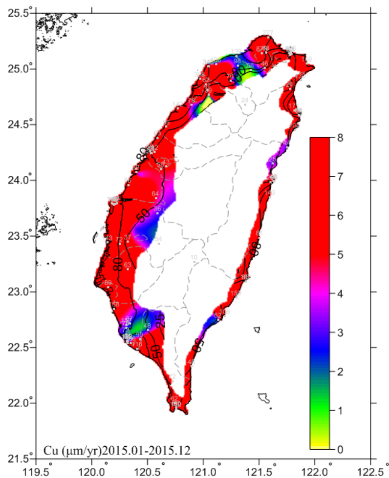
圖 6.27 2015 一年期銅腐蝕速率
