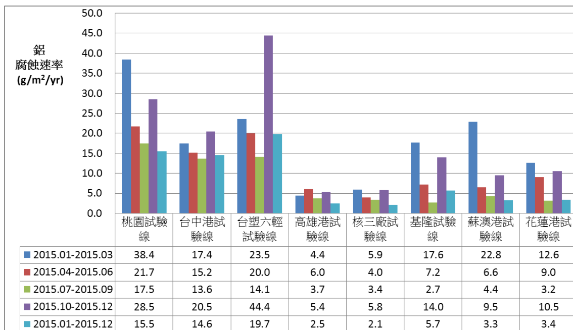
圖 6.4 垂直海岸試驗線鋁腐蝕速率比較圖
