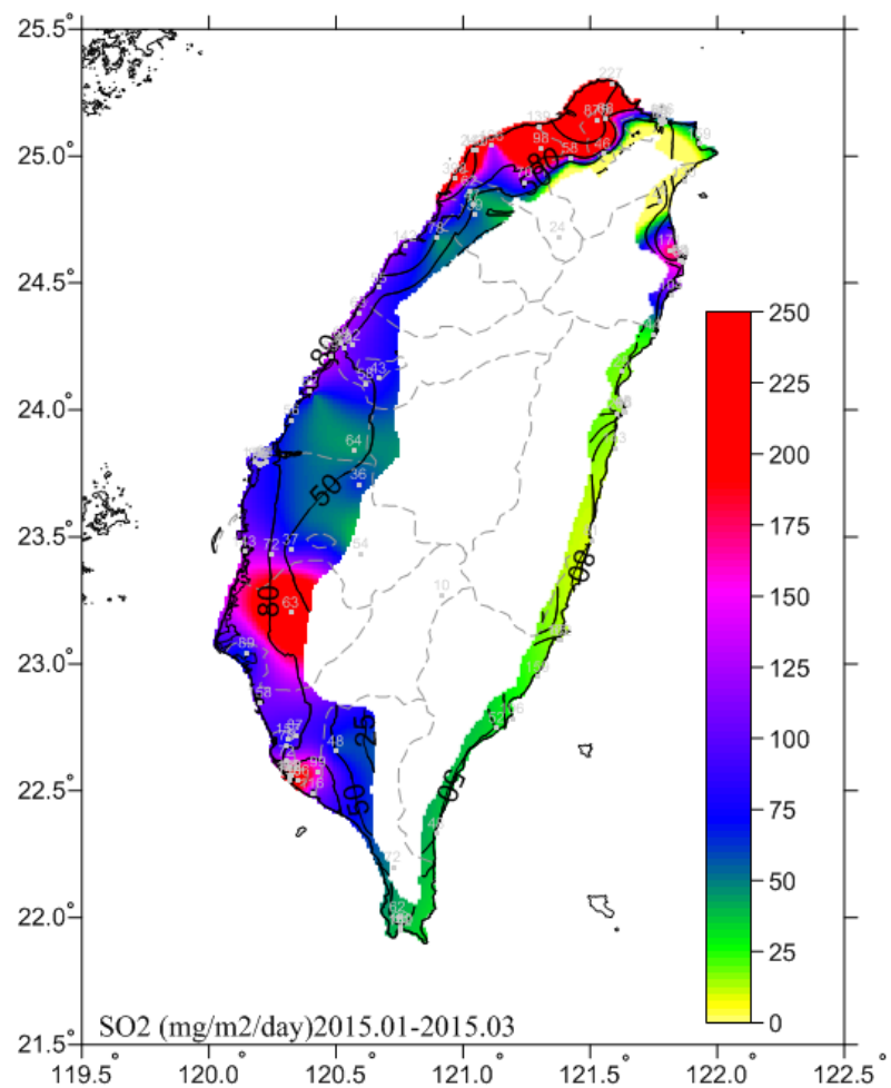
圖 5.1 2015.01-2015.03 二氧化硫沉積速率圖
