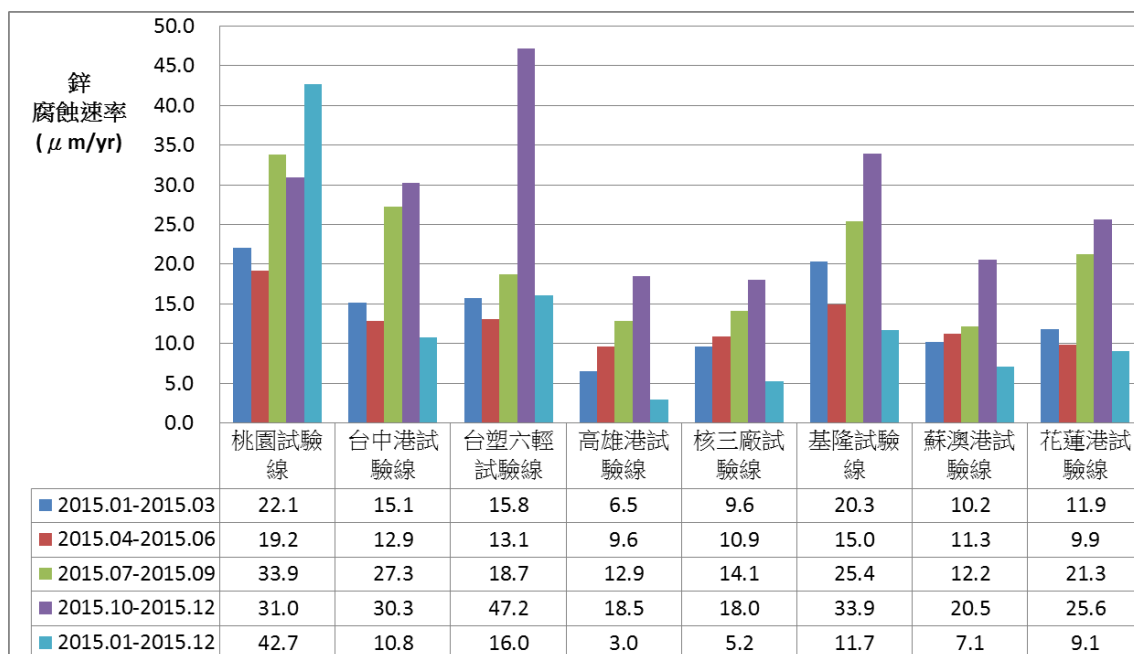
圖 6.2 垂直海岸試驗線鋅腐蝕速率比較圖
