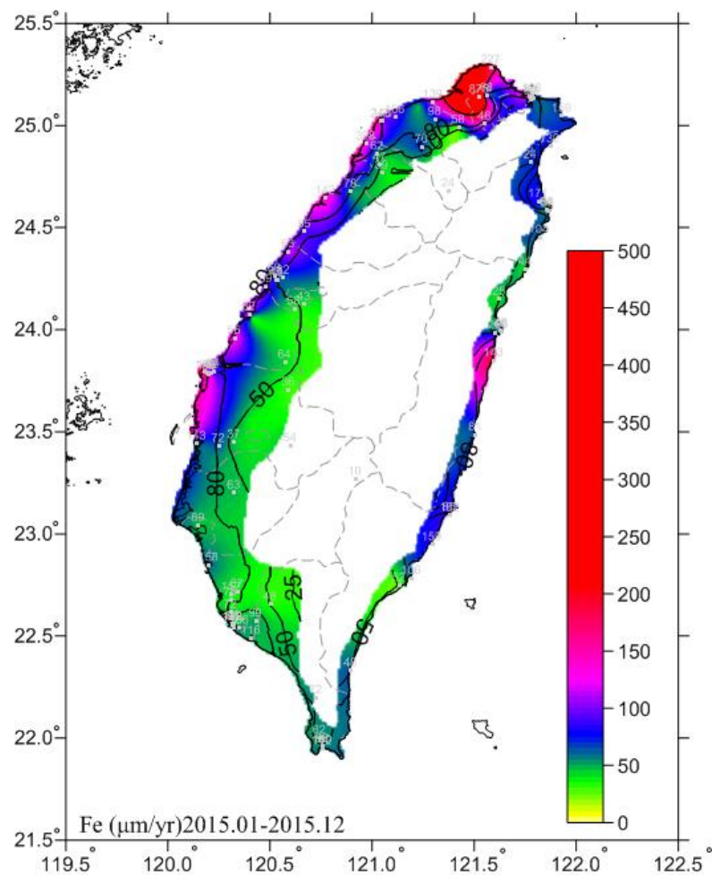
圖 6.25 2015 一年期碳鋼腐蝕速率
