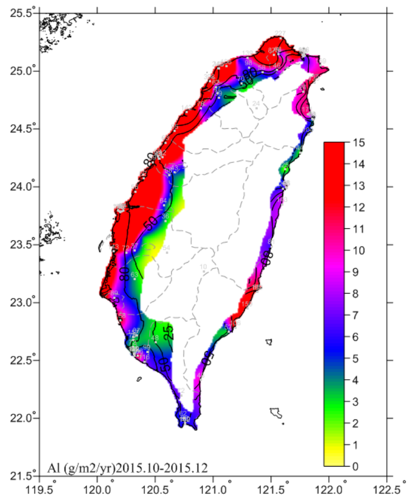
圖 6.24 2015.10-2015.12 鋁腐蝕速率圖
