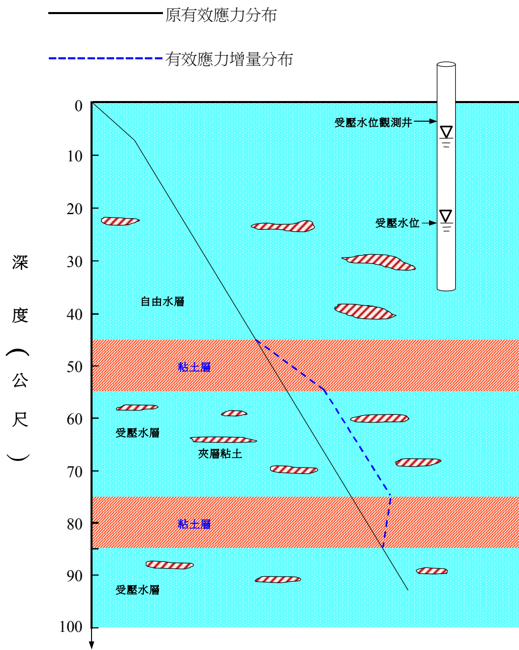
圖 2.3 受壓水位下降引致之有效應力增量分布
