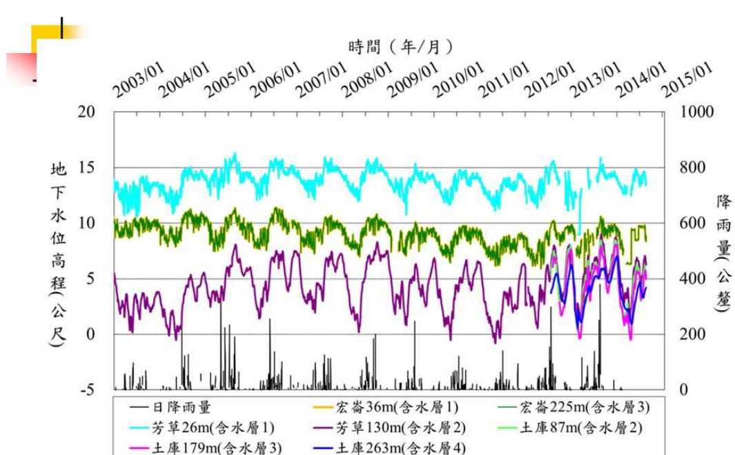
土庫國中測站分層水位變化圖(資料來源：水利署)
