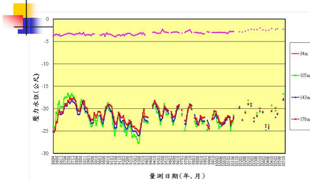
布袋港分層水位變化200m(手動量測86/04起)
