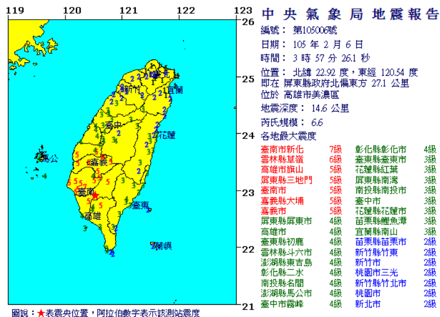
圖5.56 2016年2月6日03時57分高雄美濃地震(中央氣象局)
