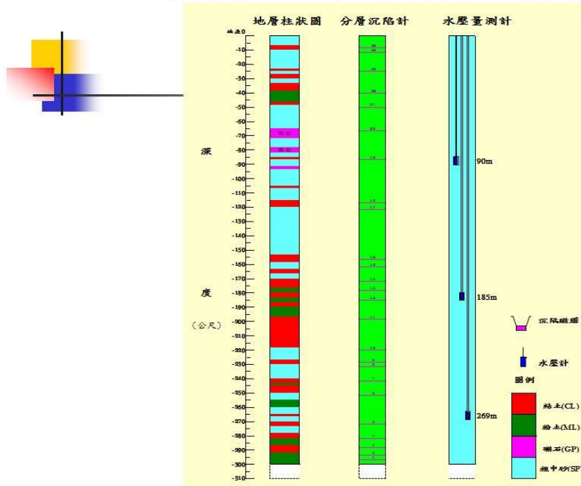
土庫國中分層沉陷及水壓量測觀測站地層柱狀圖(資料來源：水利署)
