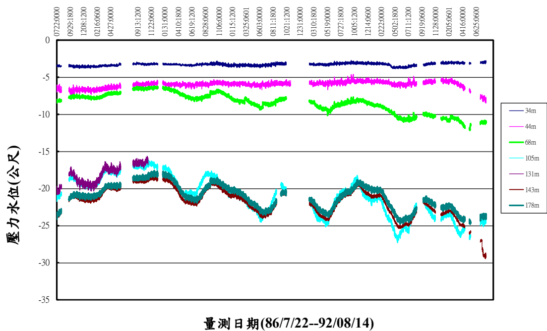
圖 4.15a 布袋港分層水位變化圖(自記式)(86/7/22-92/08/14)
