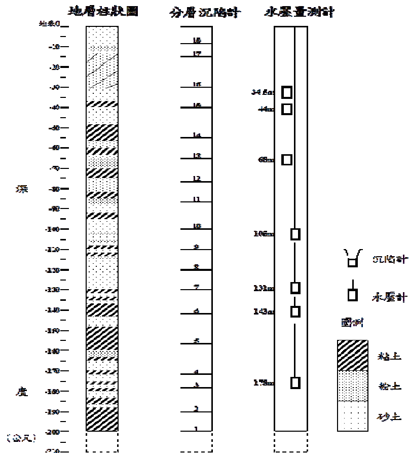
圖 4.13 布袋港分層沉陷及水壓觀測站土層柱狀圖
