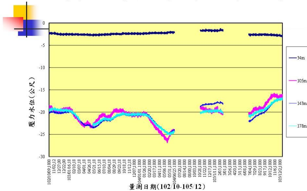
布袋港分層水位變化圖200m(自記式)
