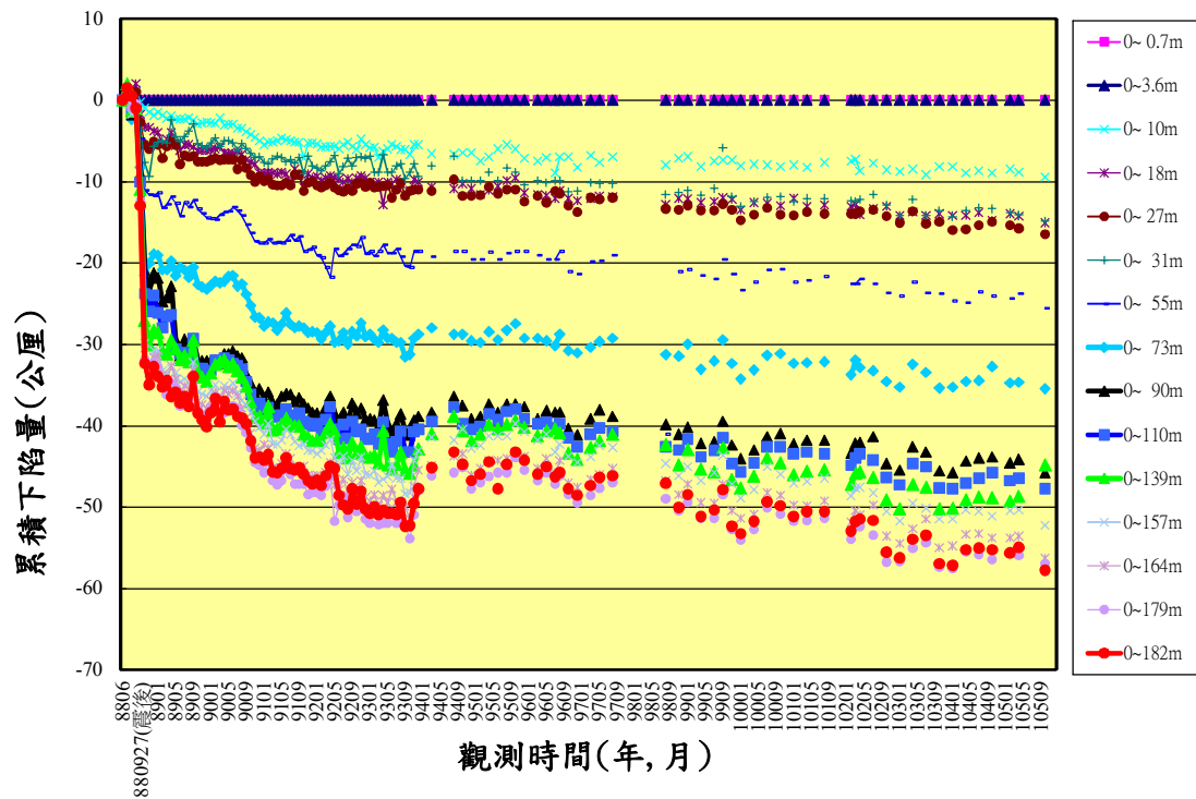
圖 4.32 臺中港分層累積下陷量圖(200m)
