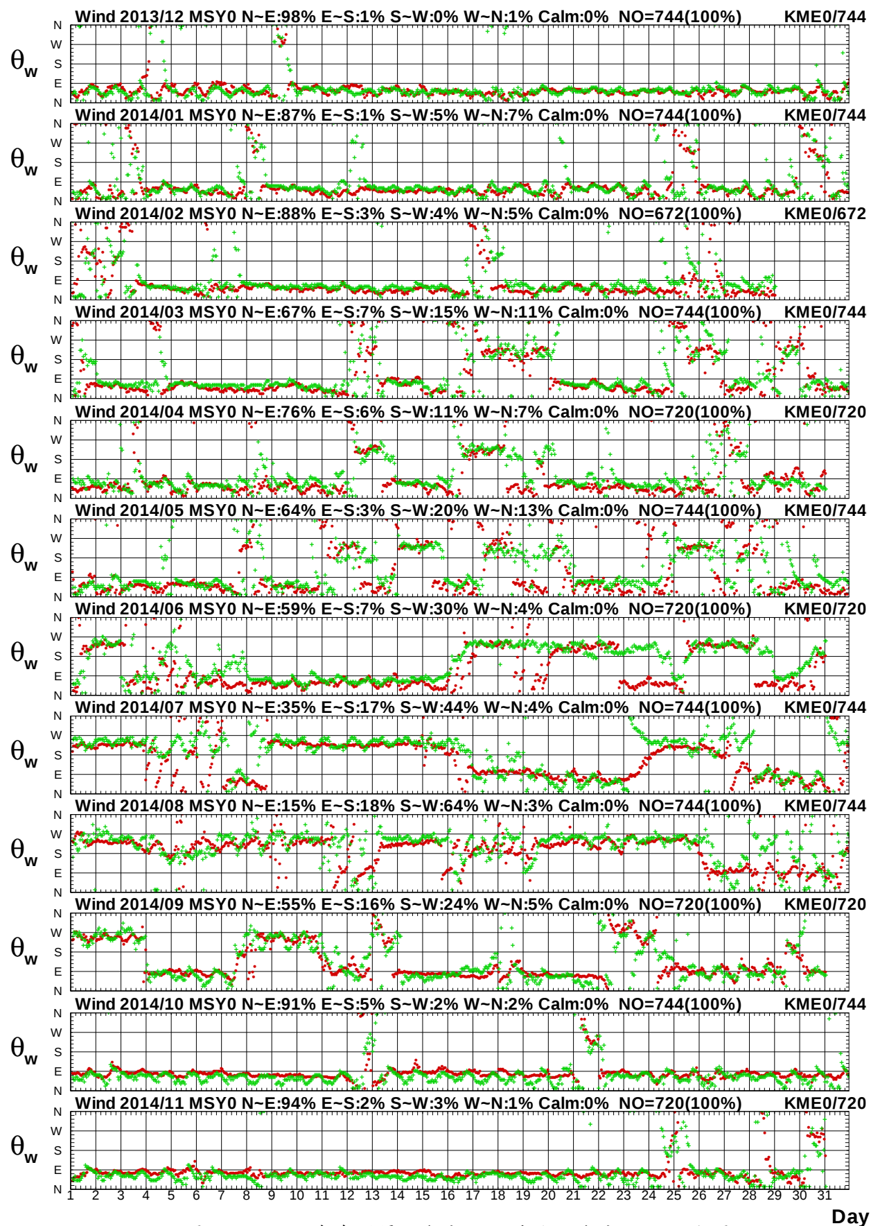
圖 1.9b 2014年每月馬祖海域 Y 站與金門海域 E 站風向圖
