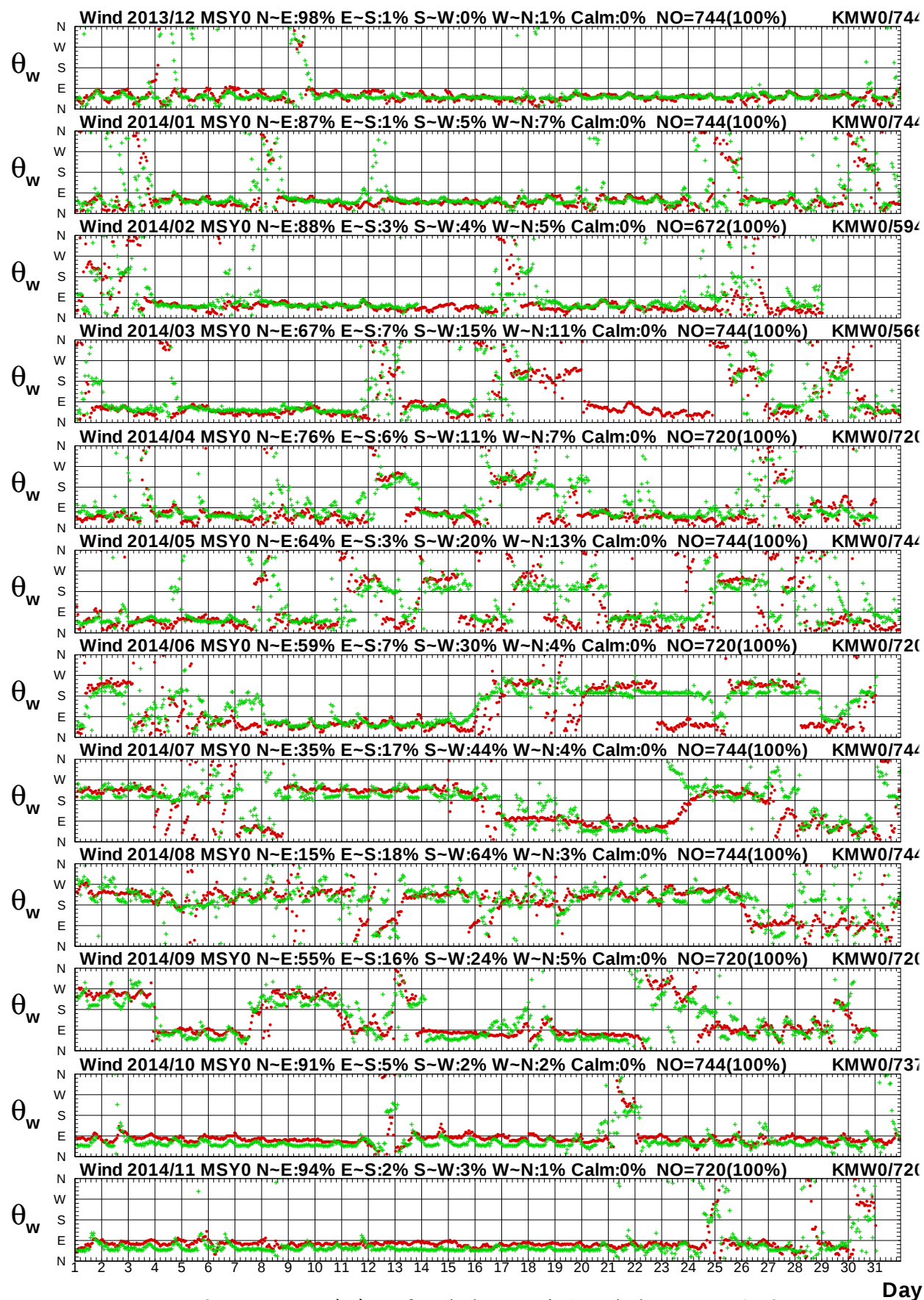
圖 1.5b 2014年每月馬祖海域 Y 站與金門海域 W 站風向圖
