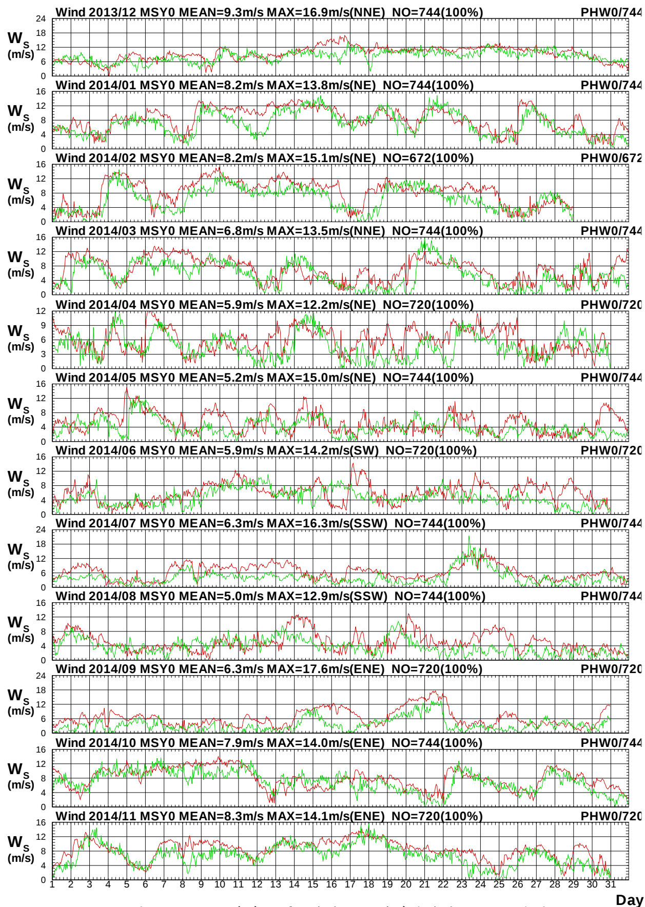
圖 1.13a 2014年每月馬祖海域 Y 站與澎湖海域 W 站風速圖
