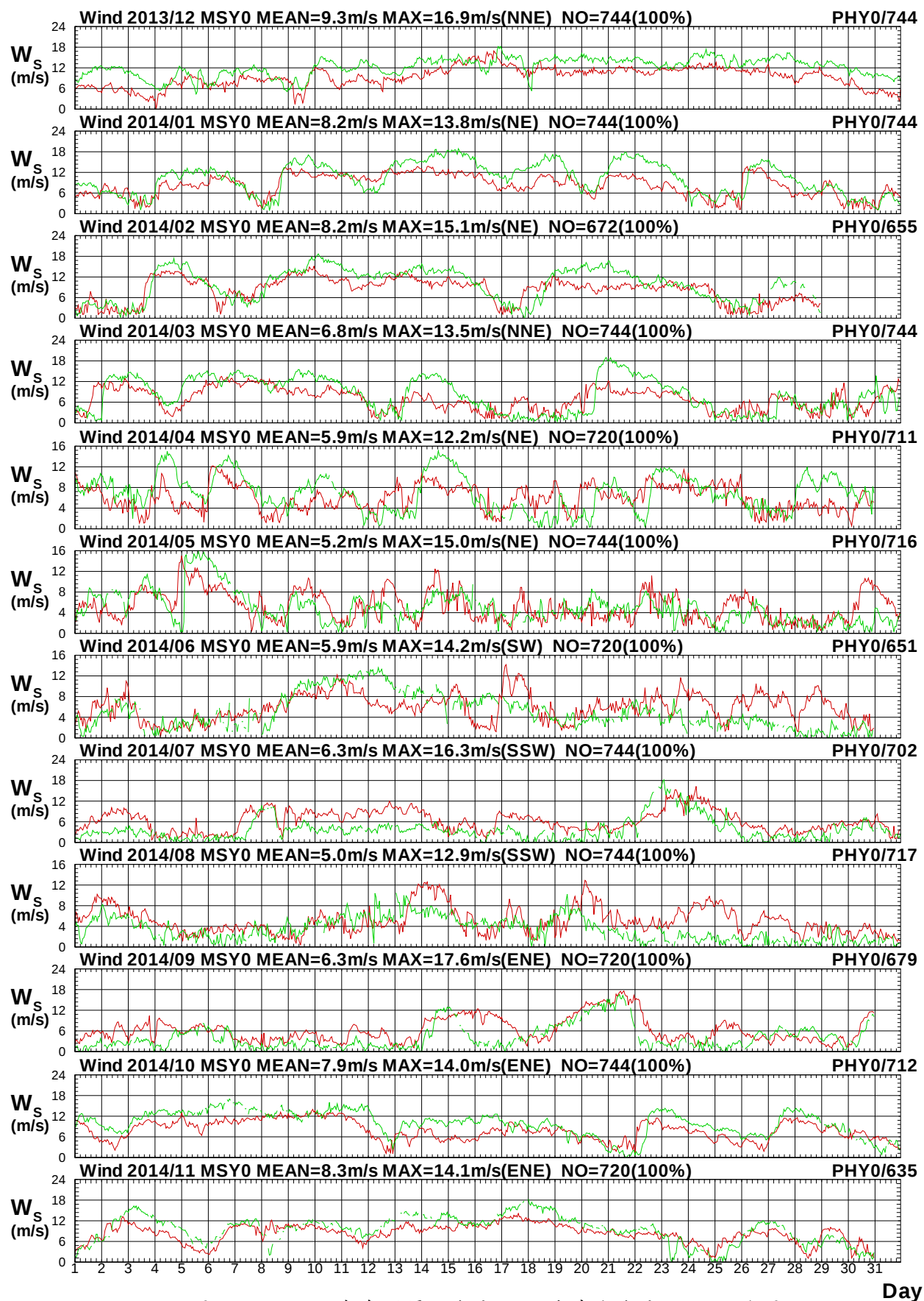
圖 1.12a 2014年每月馬祖海域 Y 站與澎湖海域 Y 站風速圖
