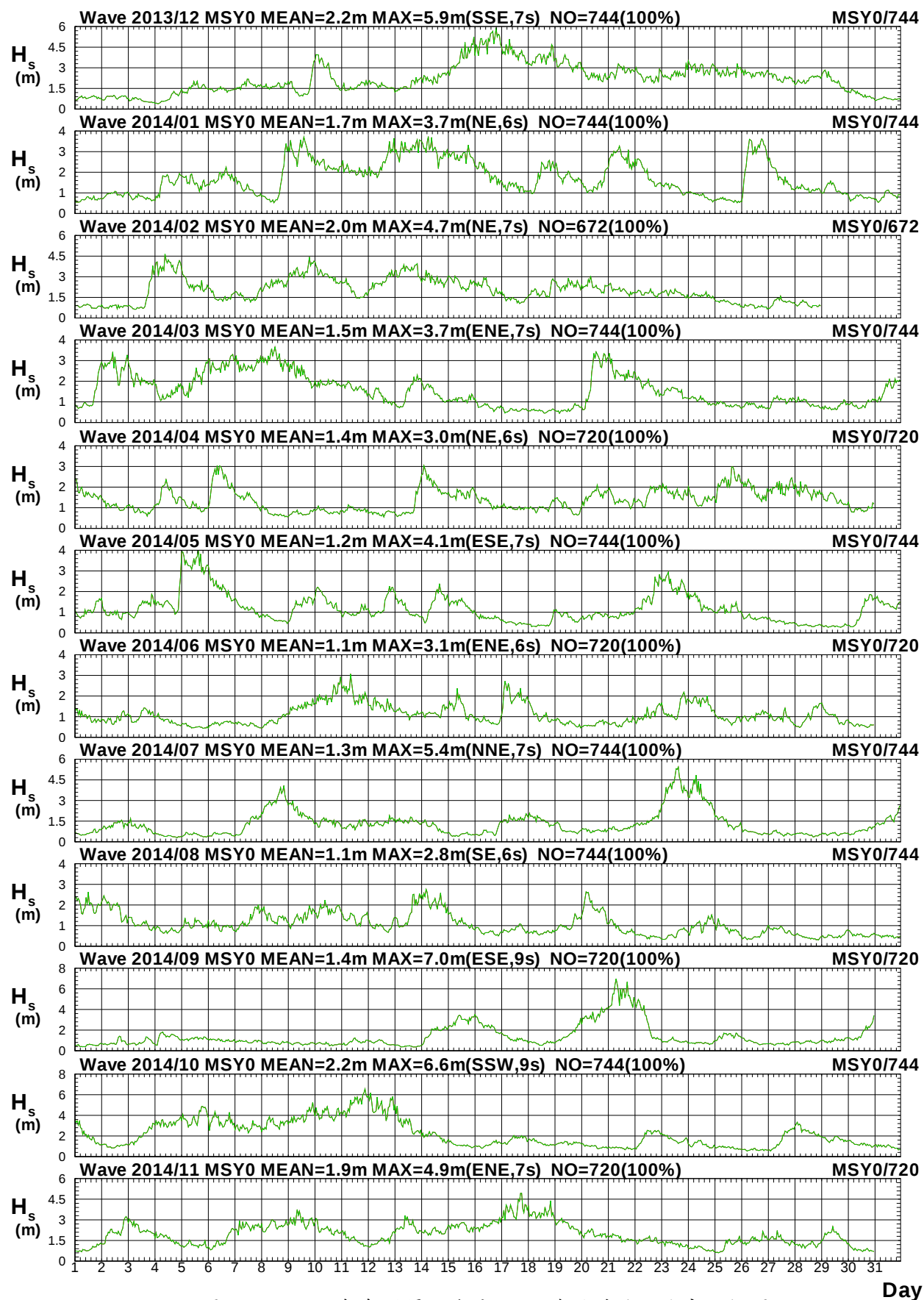
圖 2.1a 2014年每月馬祖海域 Y 站修補前後之波高比較圖
