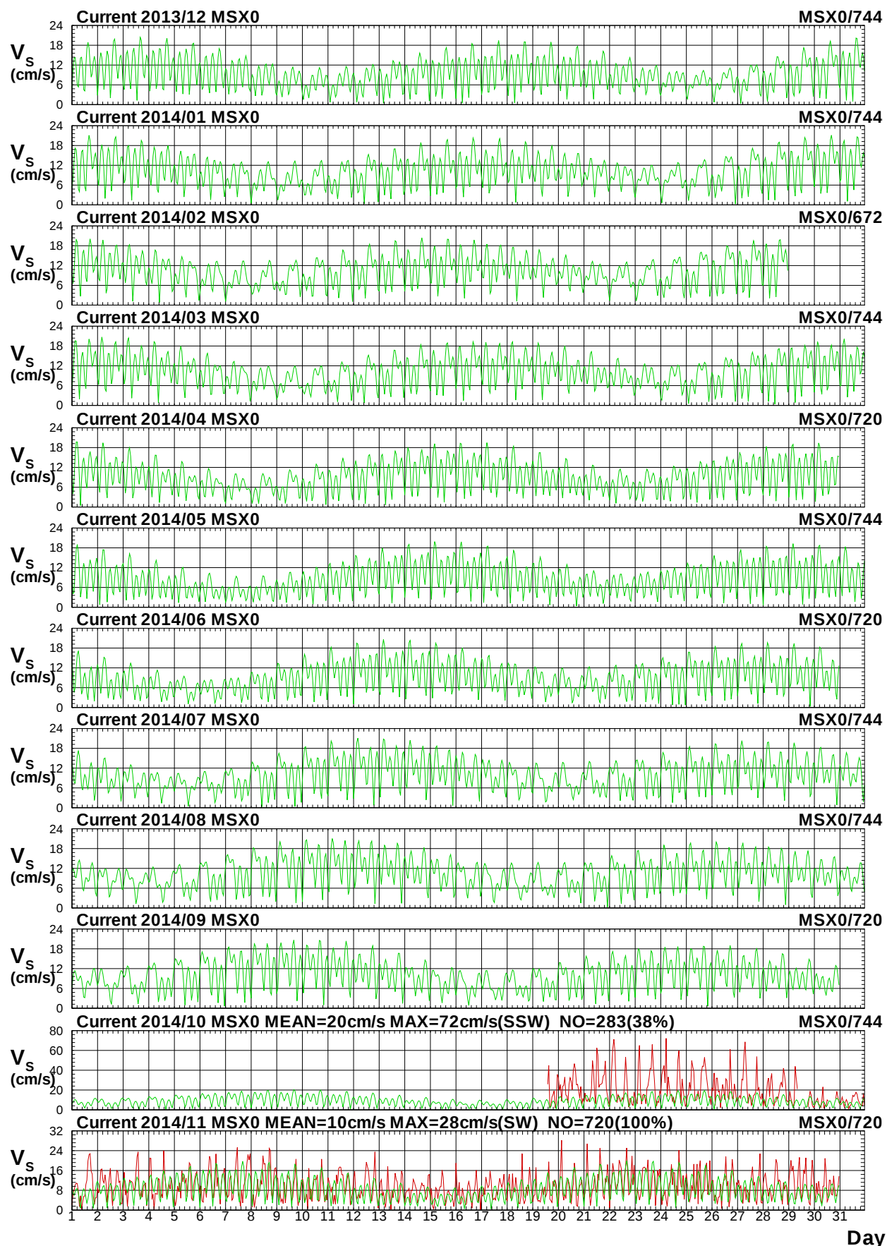
圖 4.1a 2014年每月馬祖海域 X 站觀測與潮流流速比較圖
