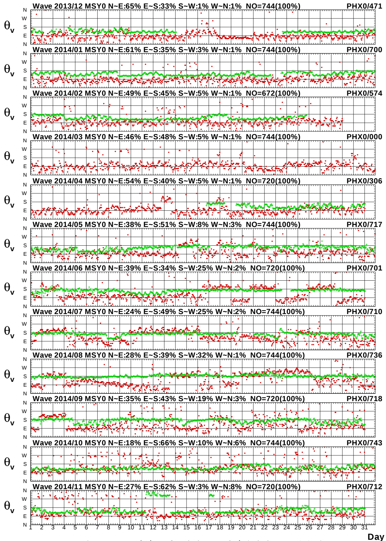
圖 2.7c 2014年每月馬祖海域 Y 站與澎湖海域 X 站波向圖
