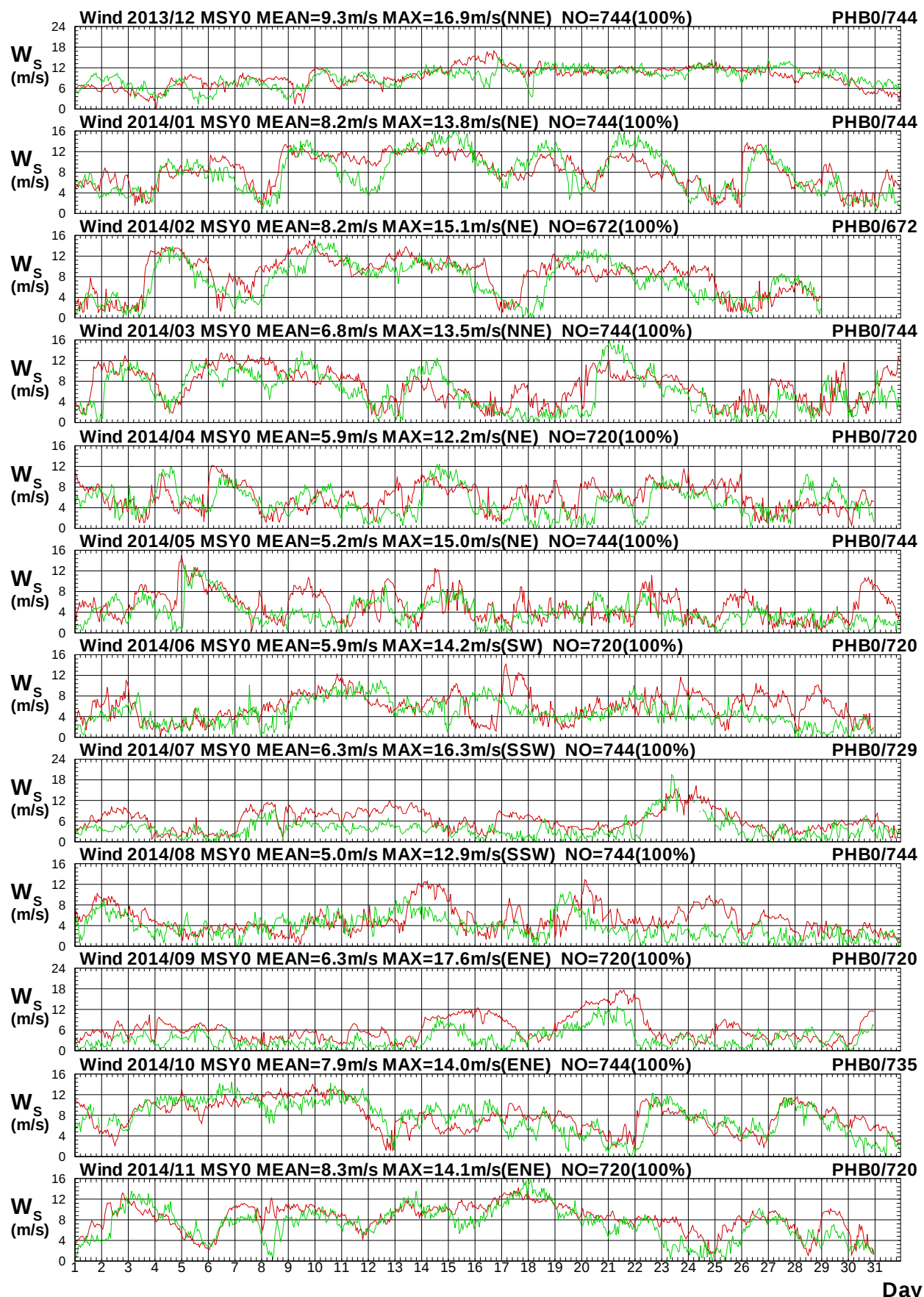
圖 1.14a 2014年每月馬祖海域 Y 站與澎湖海域 B 站風速圖
