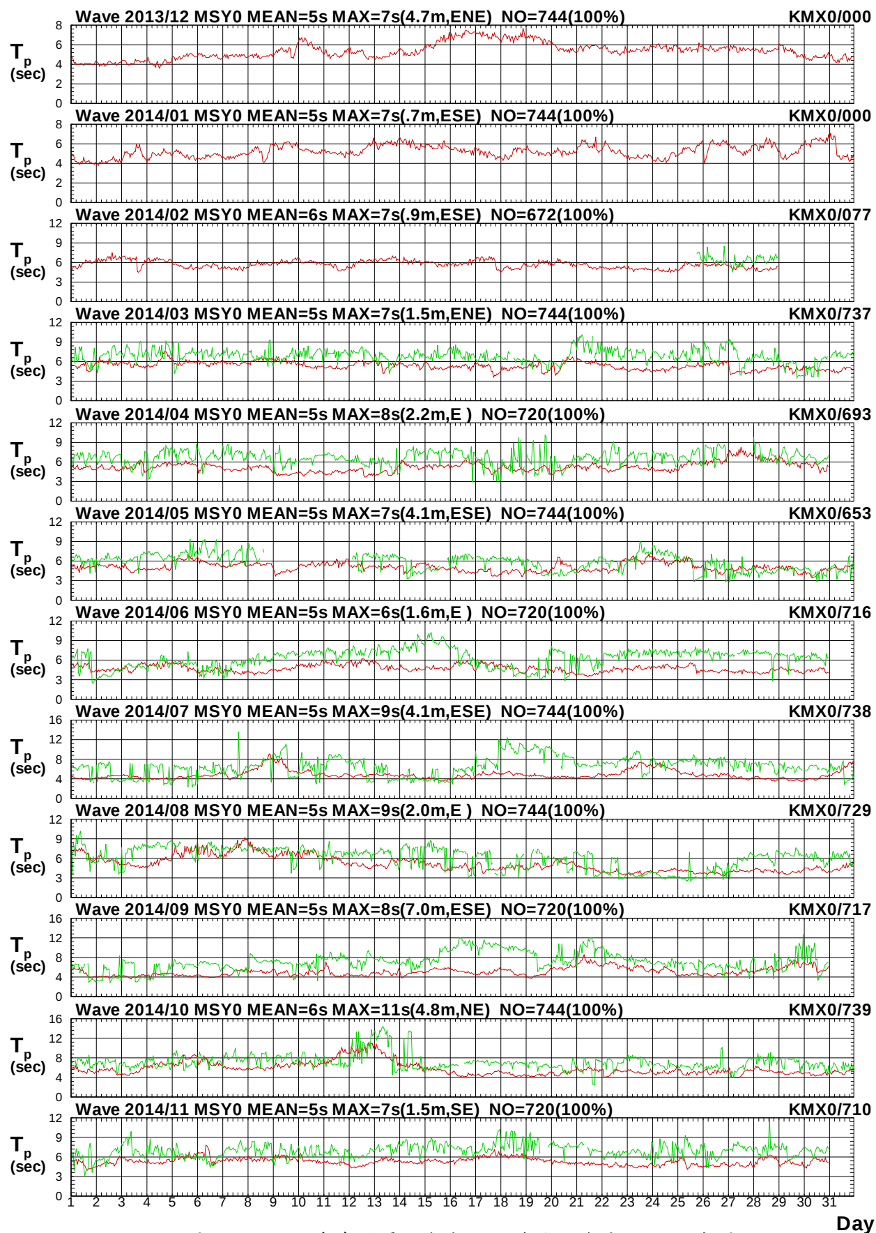
圖 2.3b 2014年每月馬祖海域 Y 站與金門海域 X 站週期圖
