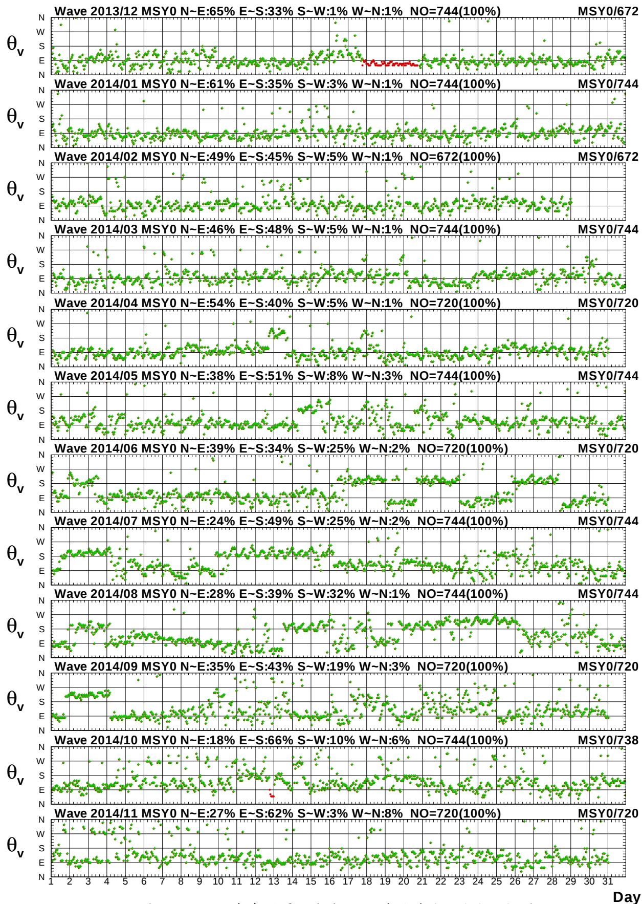
圖 2.1c 2014年每月馬祖海域 Y 站修補前後之波向比較圖
