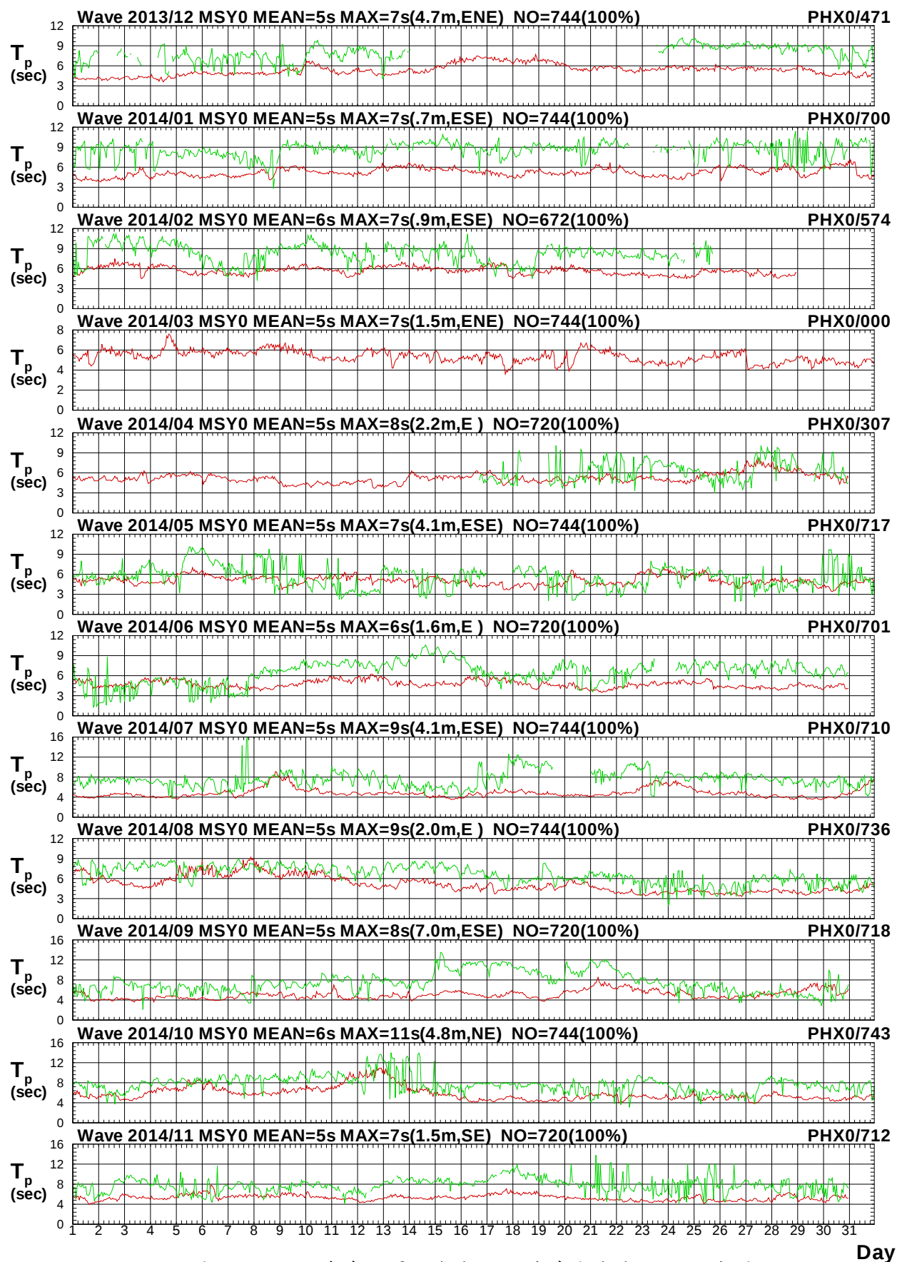
圖 2.7b 2014年每月馬祖海域 Y 站與澎湖海域 X 站週期圖
