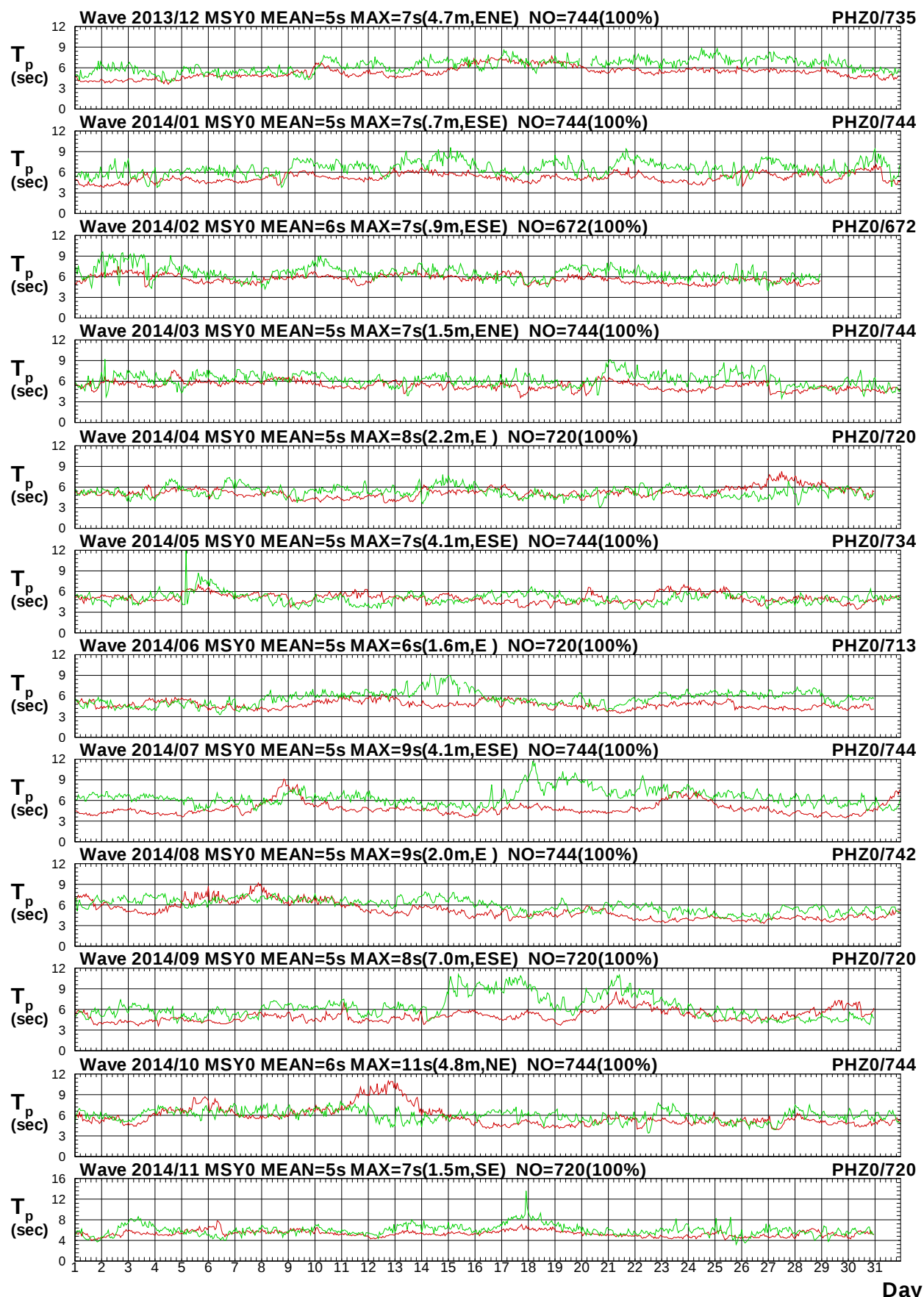
圖 2.9b 2014年每月馬祖海域 Y 站與澎湖海域 Z 站週期圖
