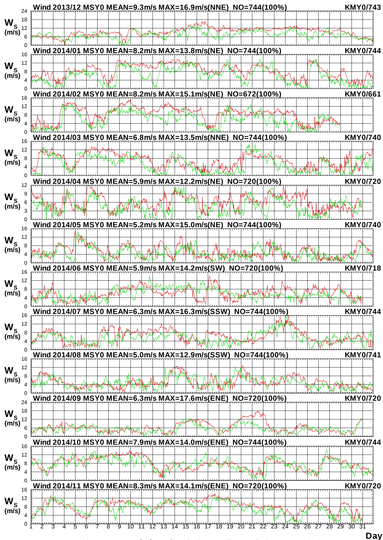
圖 1.4a 2014年每月馬祖海域 Y 站與金門海域 Y 站風速圖
