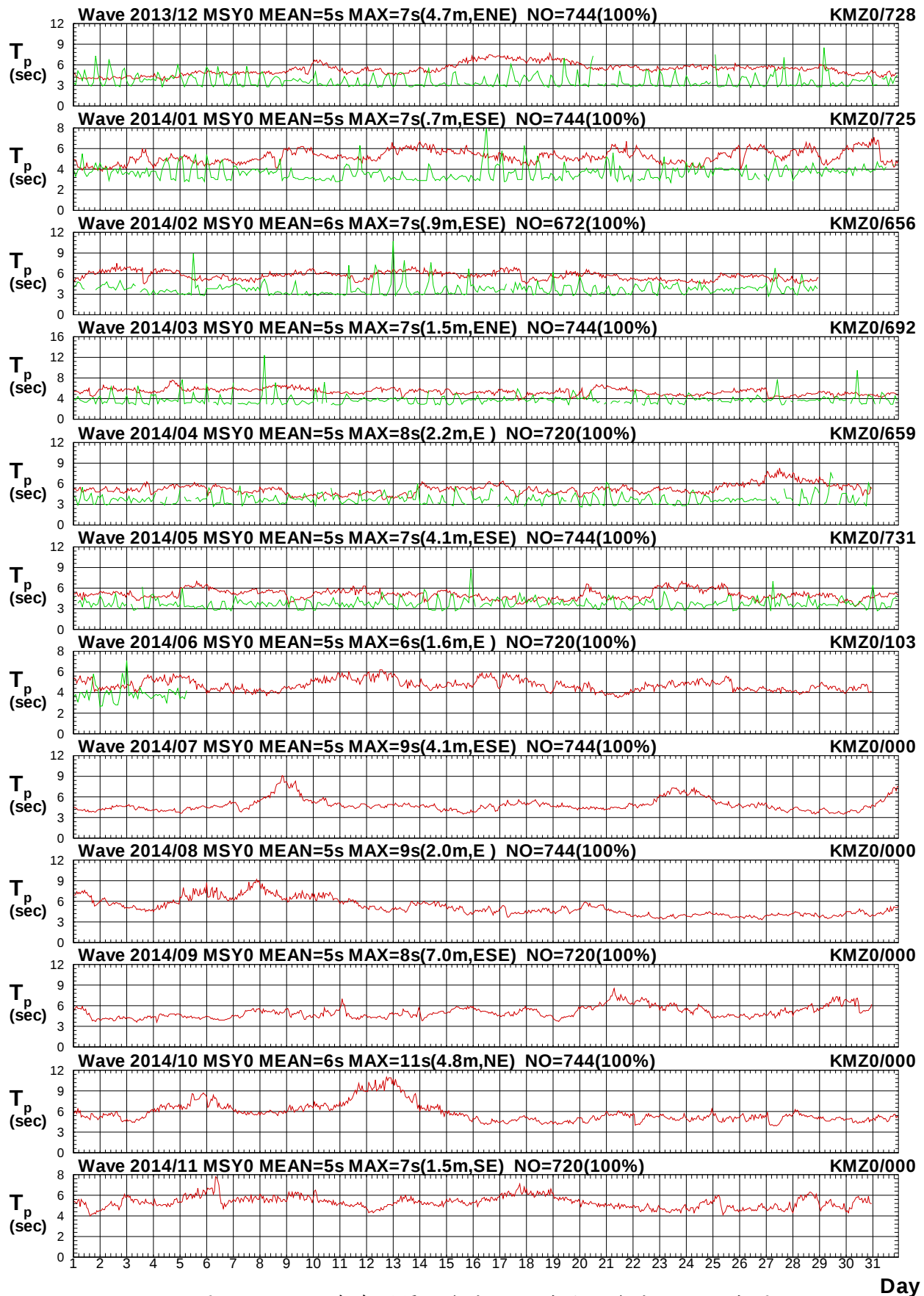
圖 2.5b 2014年每月馬祖海域 Y 站與金門海域 Z 站週期圖
