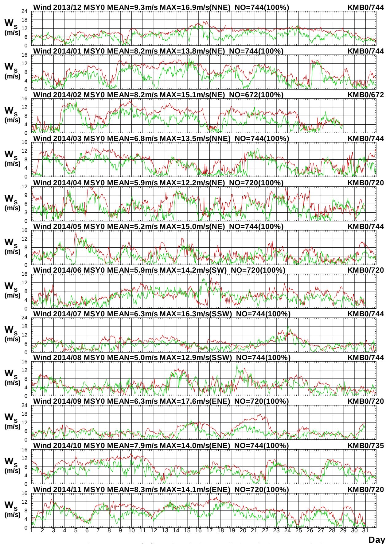
圖 1.6a 2014年每月馬祖海域 Y 站與金門海域 B 站風速圖
