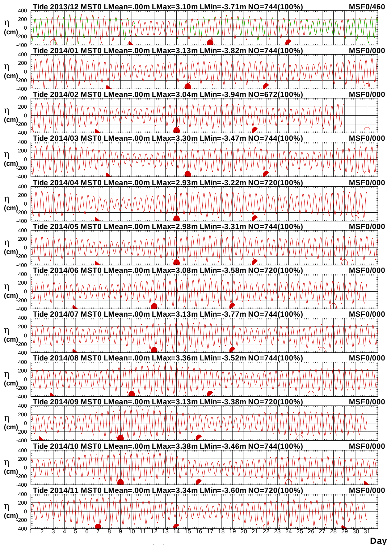
圖3.1.3 2014年每月馬祖海域 T 站與 F 站潮位比較圖
