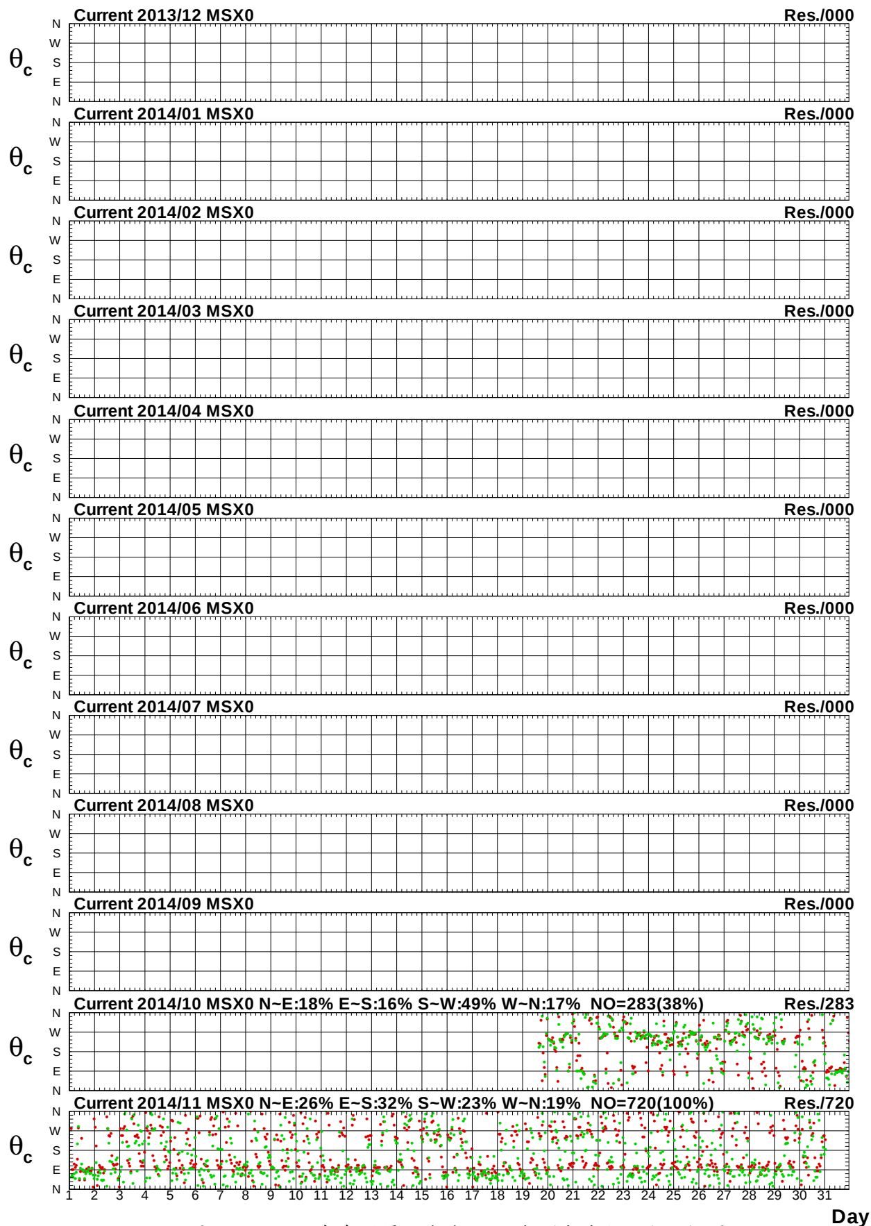
圖 4.2b 2014 年每月馬祖海域 X 站觀測與非潮流向比較圖
