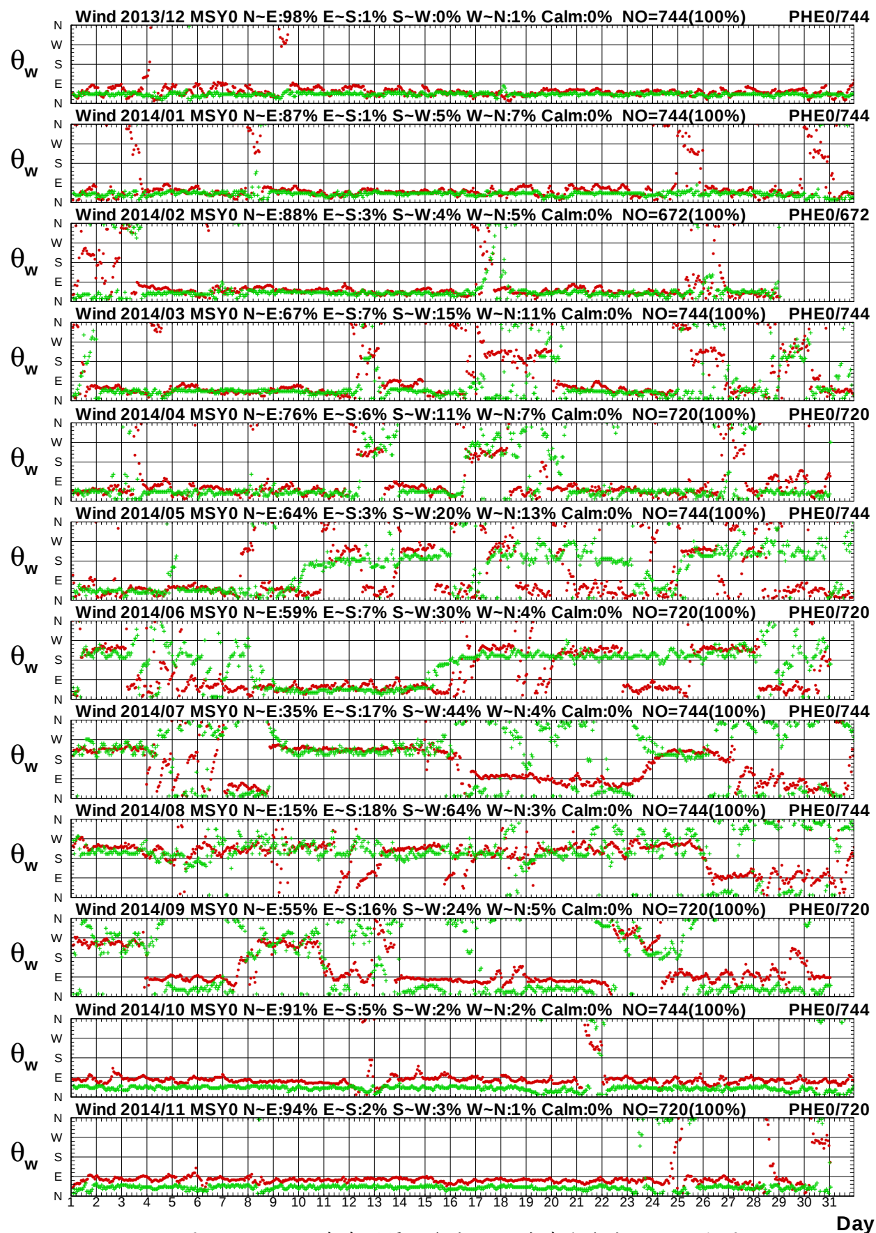
圖 1.15b 2014年每月馬祖海域 Y 站與澎湖海域 E 站風向圖
