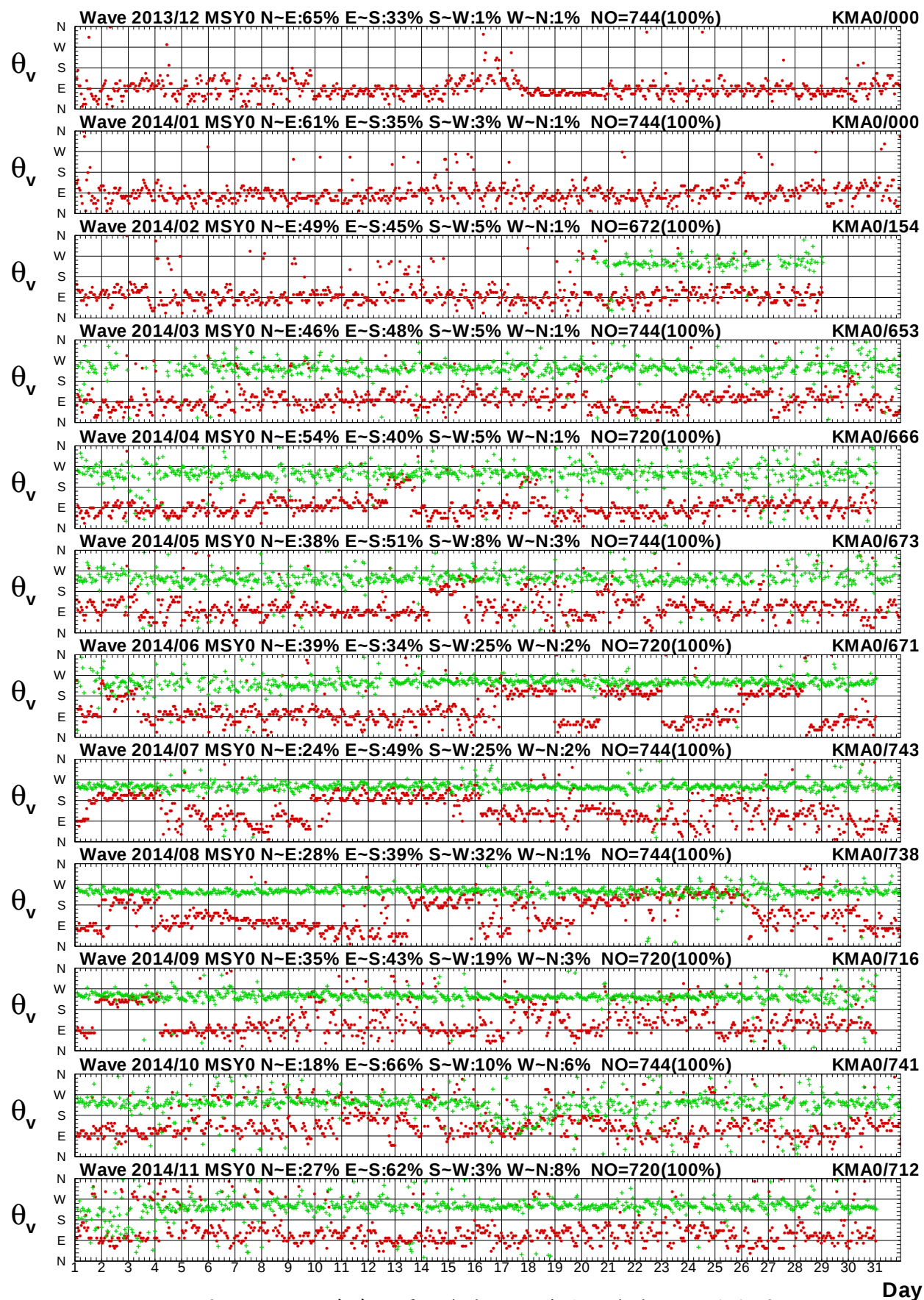
圖 2.6c 2014年每月馬祖海域 Y 站與金門海域 A 站波向圖
