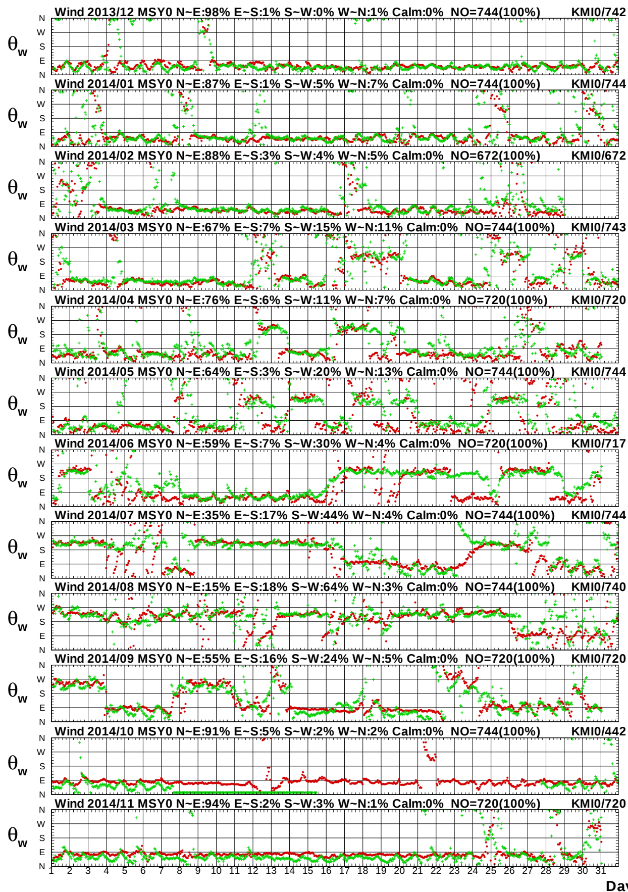
圖 1.11b 2014年每月馬祖海域 Y 站與金門海域 I 站風向圖
