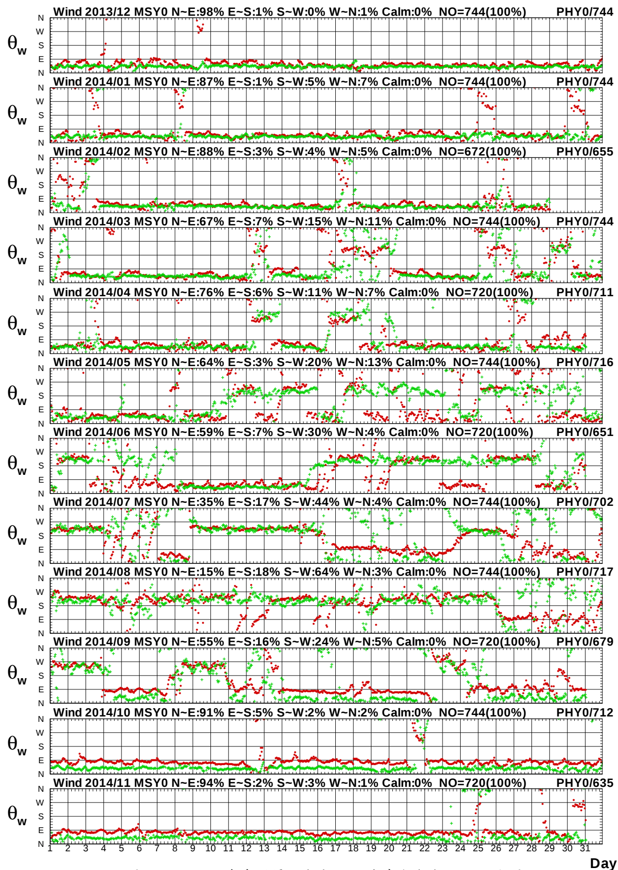
圖 1.12b 2014年每月馬祖海域 Y 站與澎湖海域 Y 站風向圖
