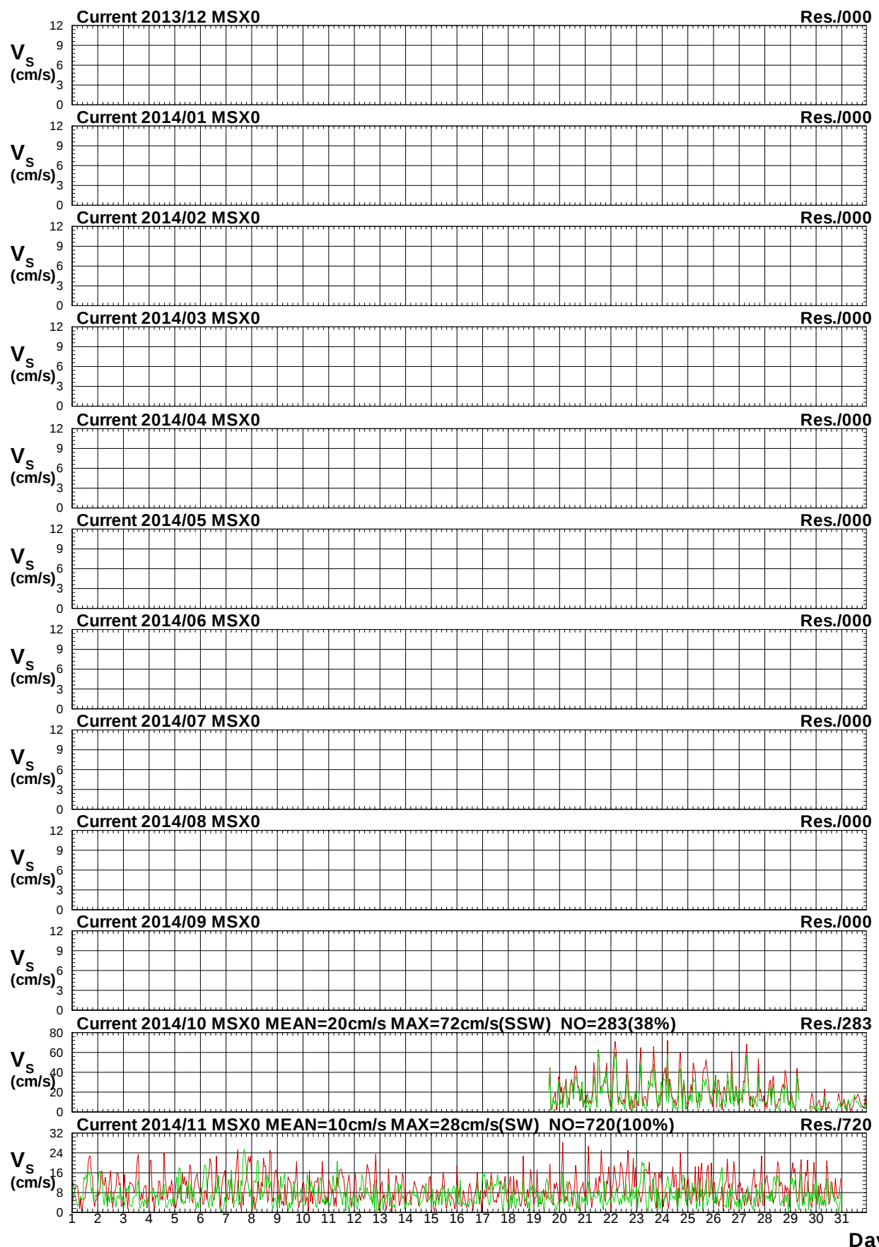
圖 4.2a 2014年每月馬祖海域 X 站觀測與非潮流速比較圖
