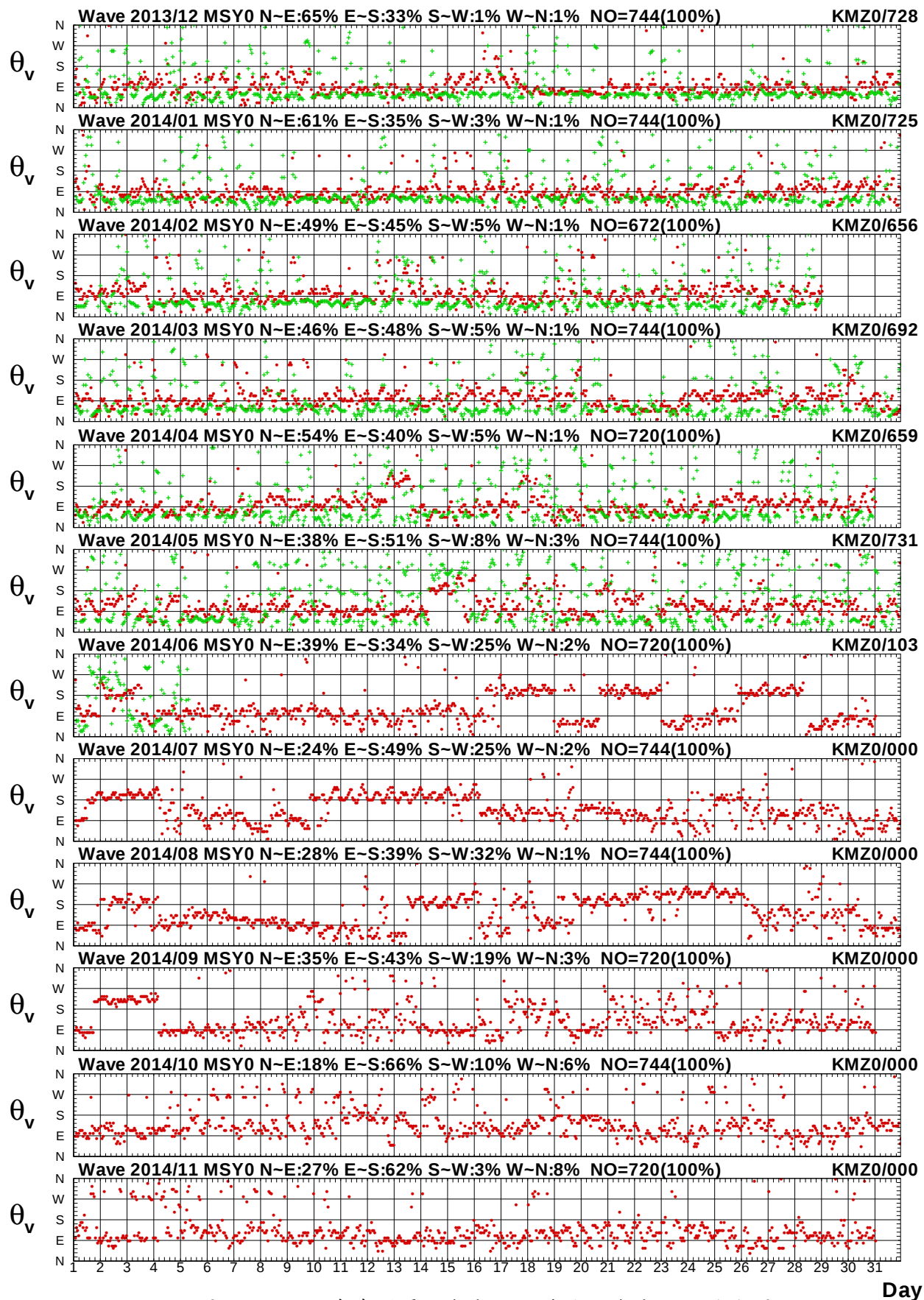
圖 2.5c 2014年每月馬祖海域 Y 站與金門海域 Z 站波向圖
