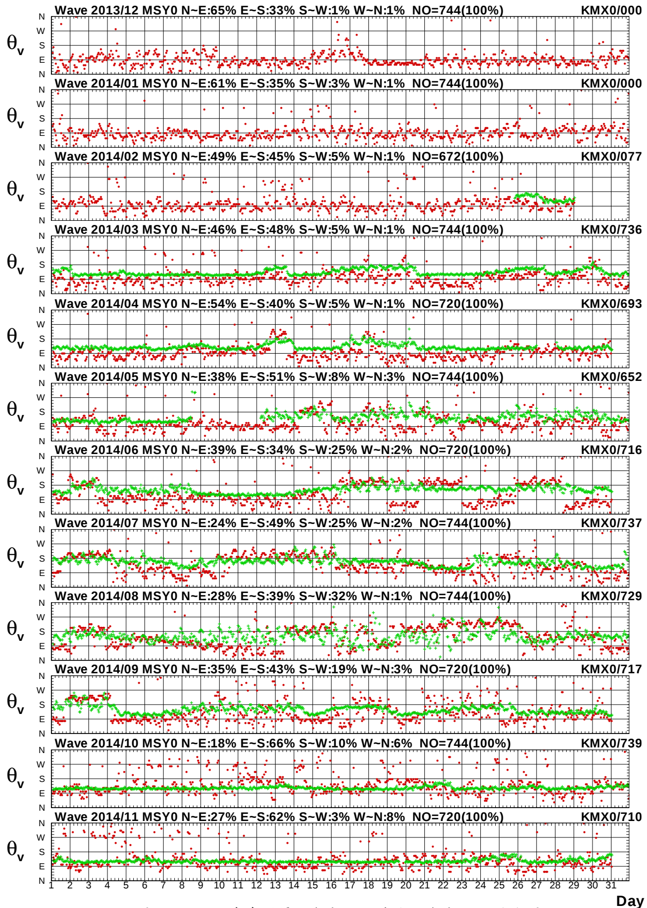
圖 2.3c 2014年每月馬祖海域 Y 站與金門海域 X 站波向圖
