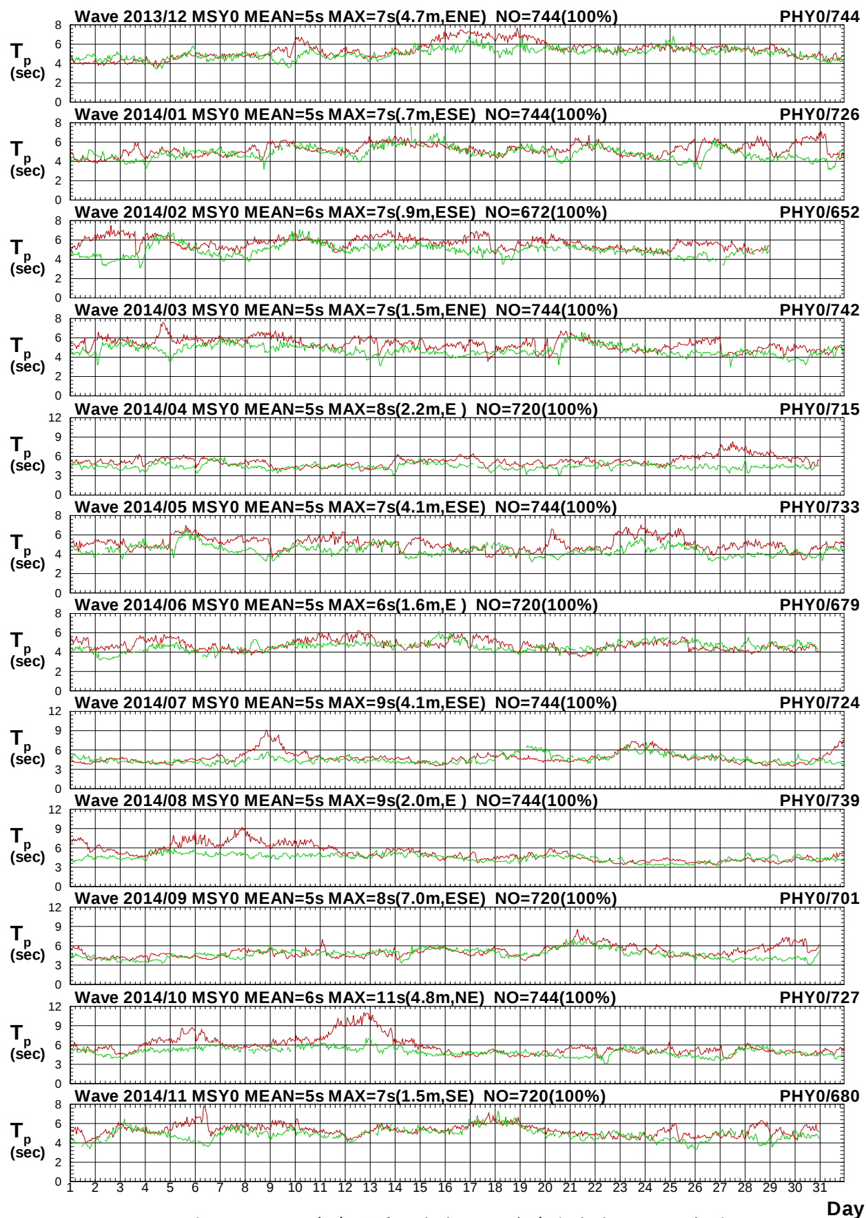
圖 2.8b 2014年每月馬祖海域 Y 站與澎湖海域 Y 站週期圖
