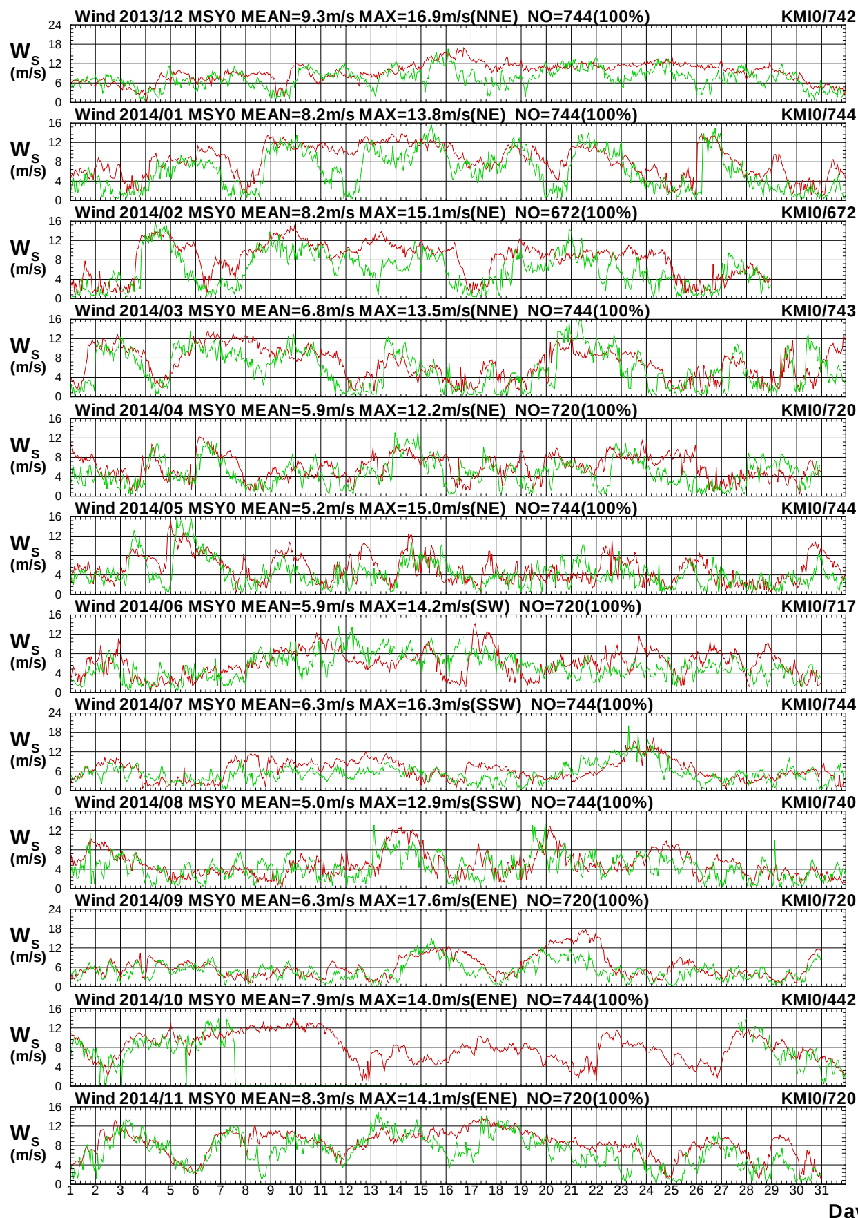
圖 1.11a 2014年每月馬祖海域 Y 站與金門海域 I 站風速圖
