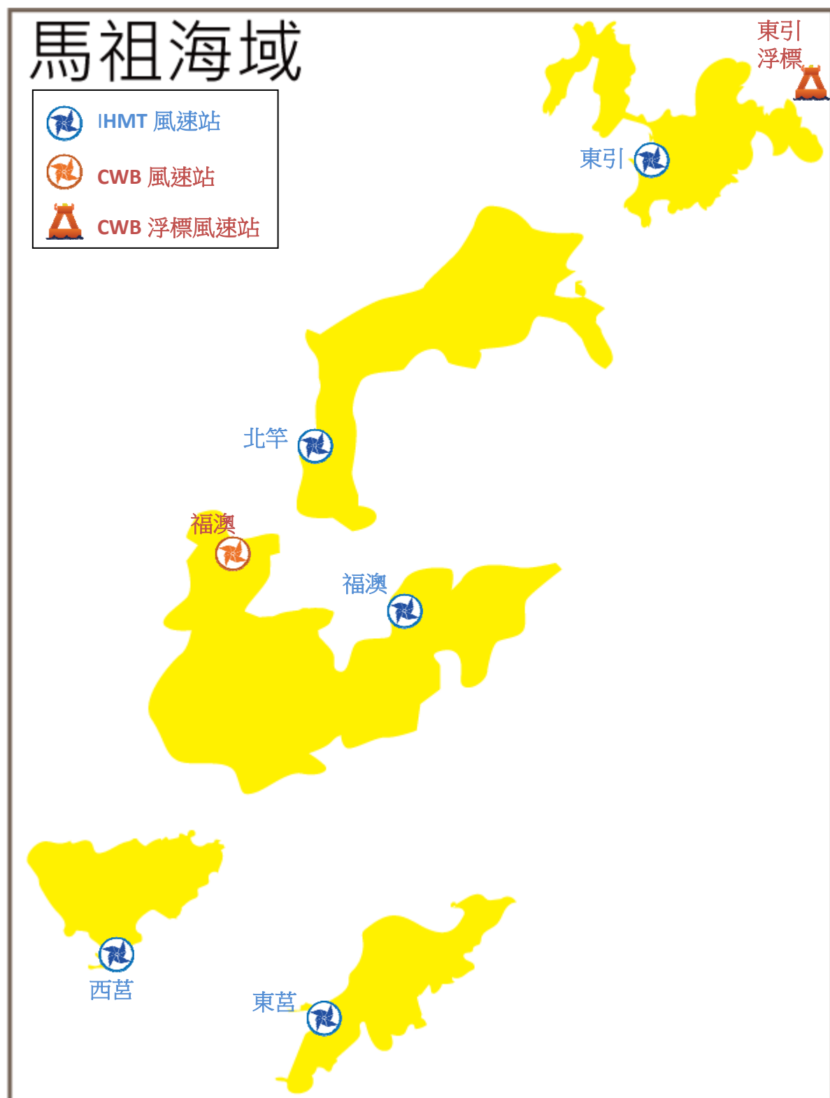
圖 1 馬祖海域風力觀測站位置示意圖
