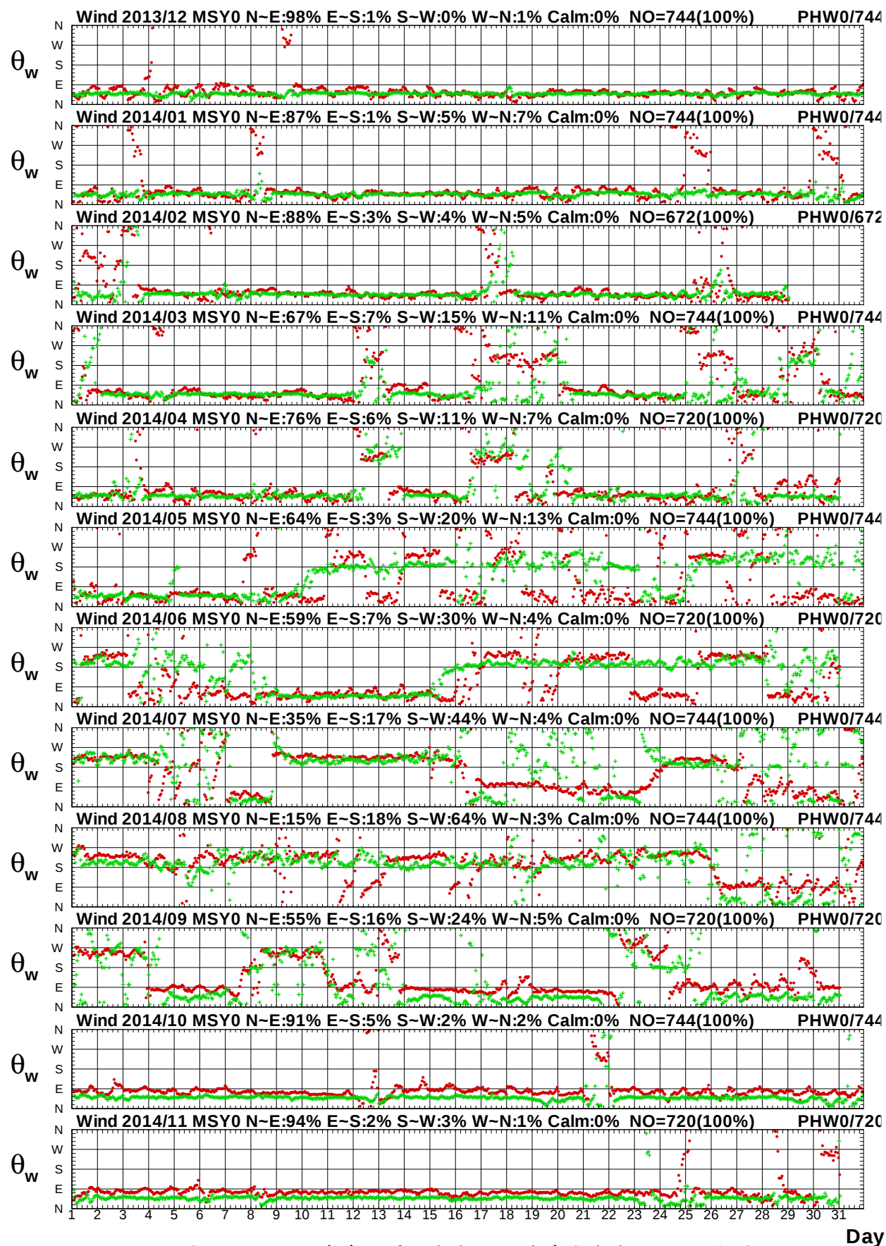
圖 1.13b 2014年每月馬祖海域 Y 站與澎湖海域 W 站風向圖
