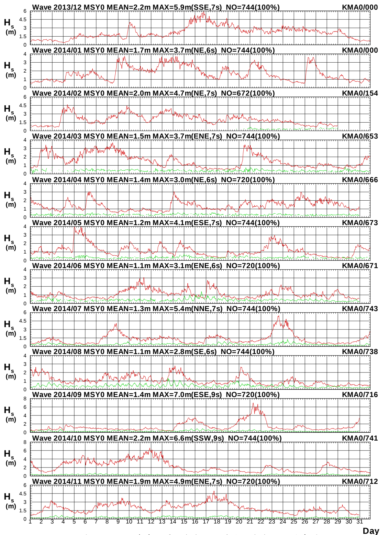
圖 2.6a 2014年每月馬祖海域 Y 站與金門海域 A 站波高圖
