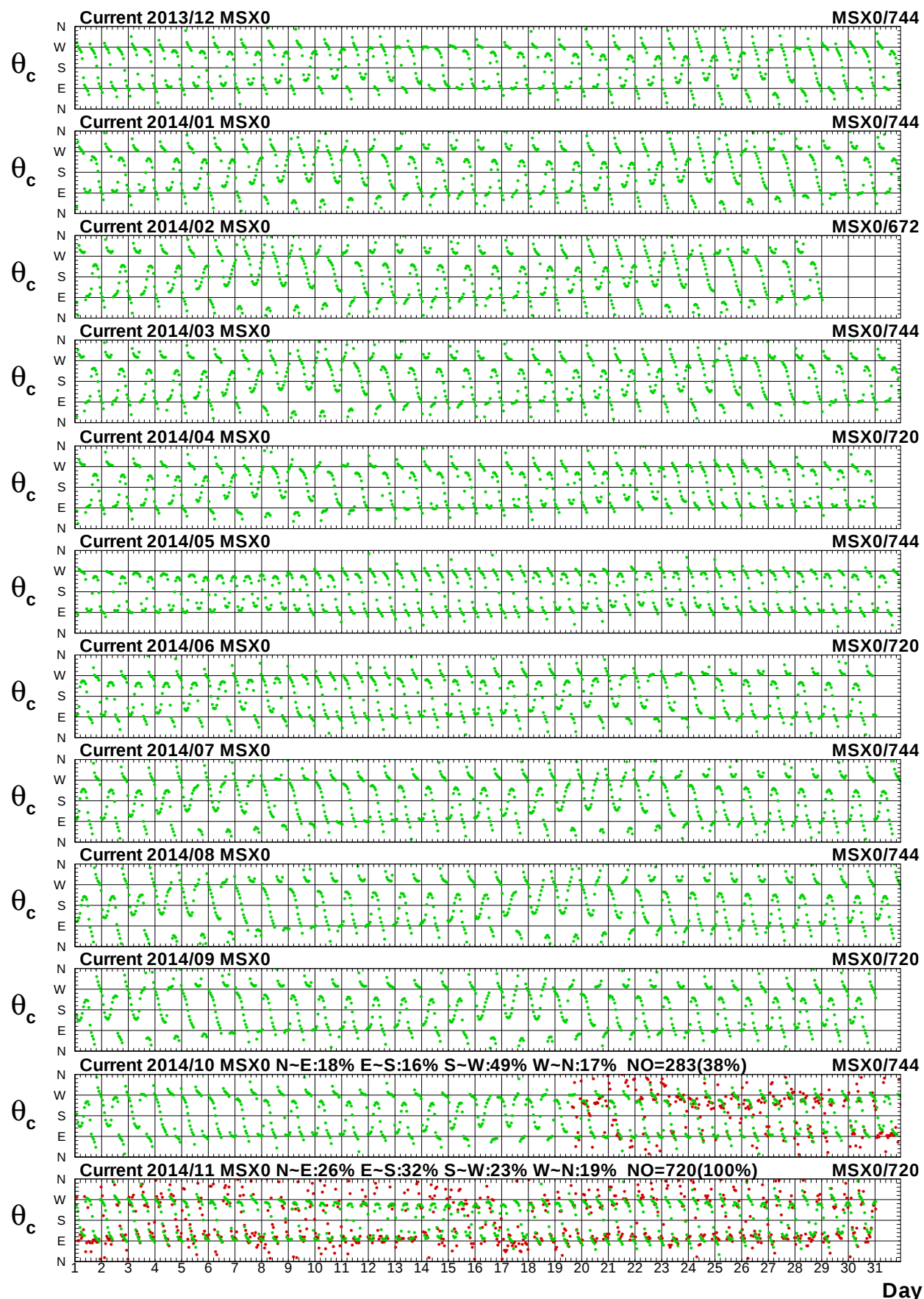
圖 4.1b 2014 年每月馬祖海域 X 站觀測與潮流流向比較圖
