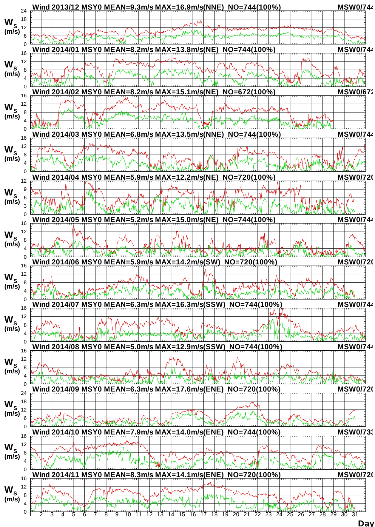
圖 1.2a 2014年每月馬祖海域 Y 站與 W 站風速比較圖
