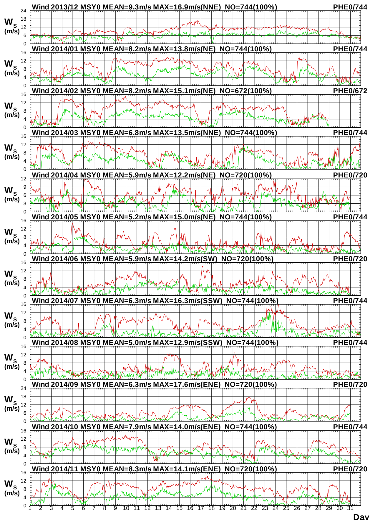
圖 1.15a 2014年每月馬祖海域 Y 站與澎湖海域 E 站風速圖
