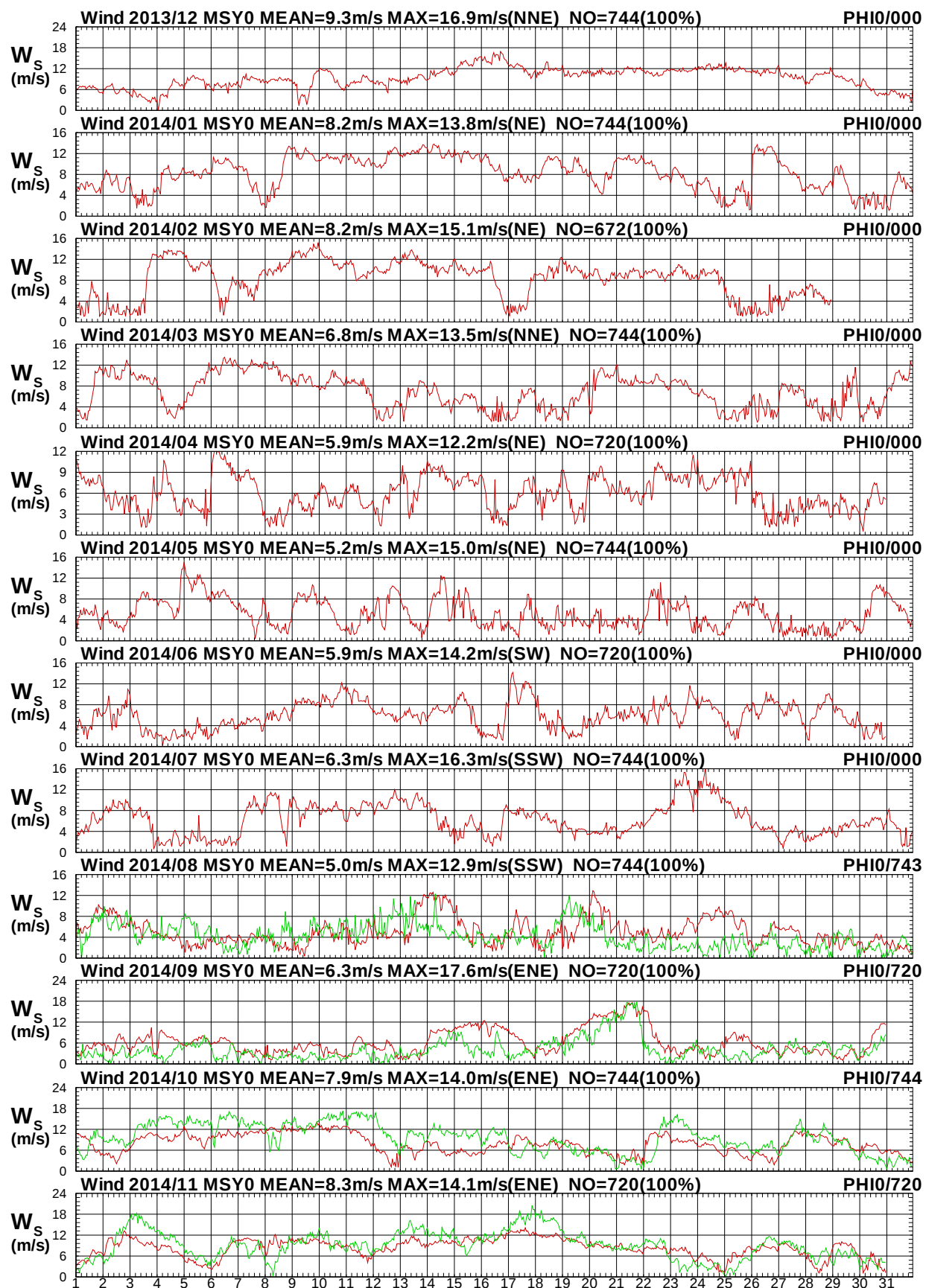
圖 1.17a 2014年每月馬祖海域 Y 站與澎湖海域 I 站風速圖
