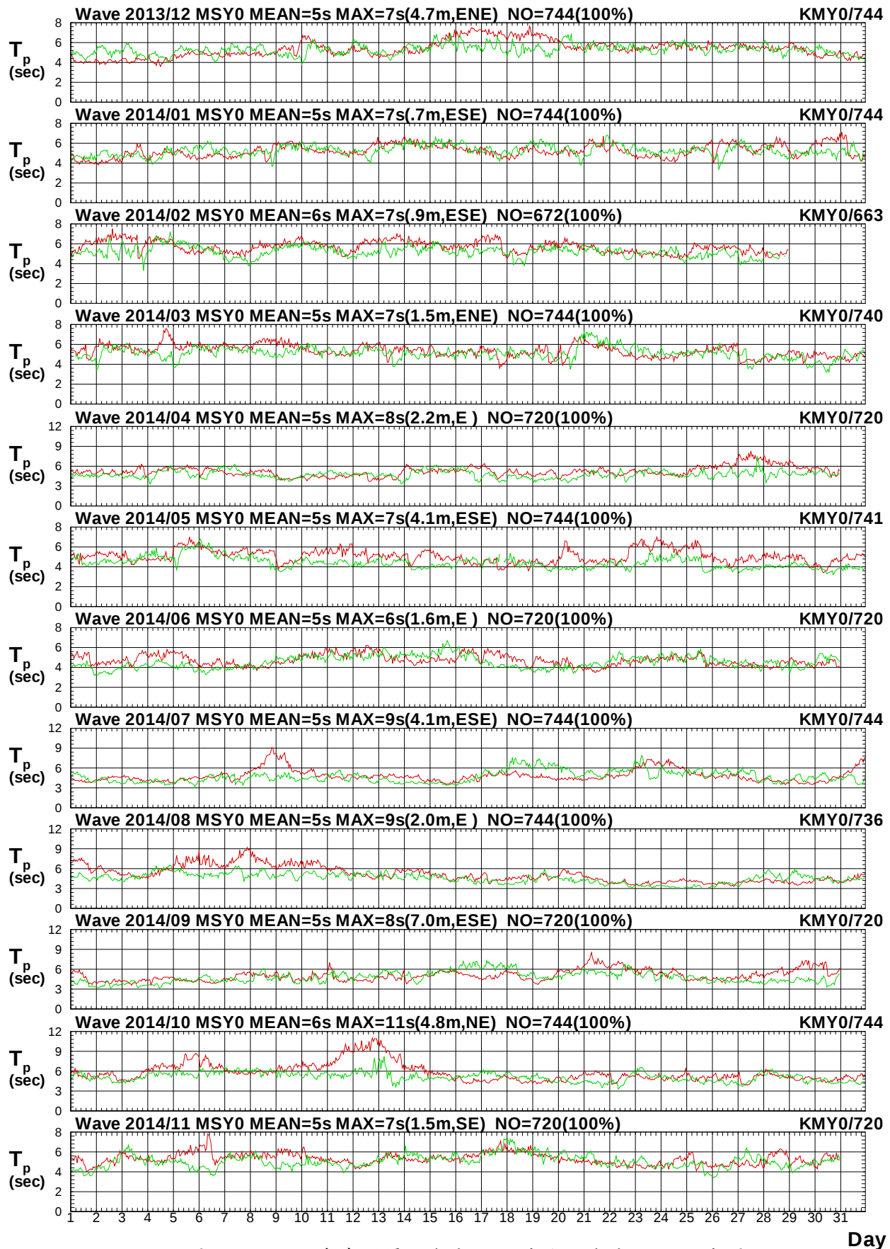
圖 2.4b 2014年每月馬祖海域 Y 站與金門海域 Y 站週期圖
