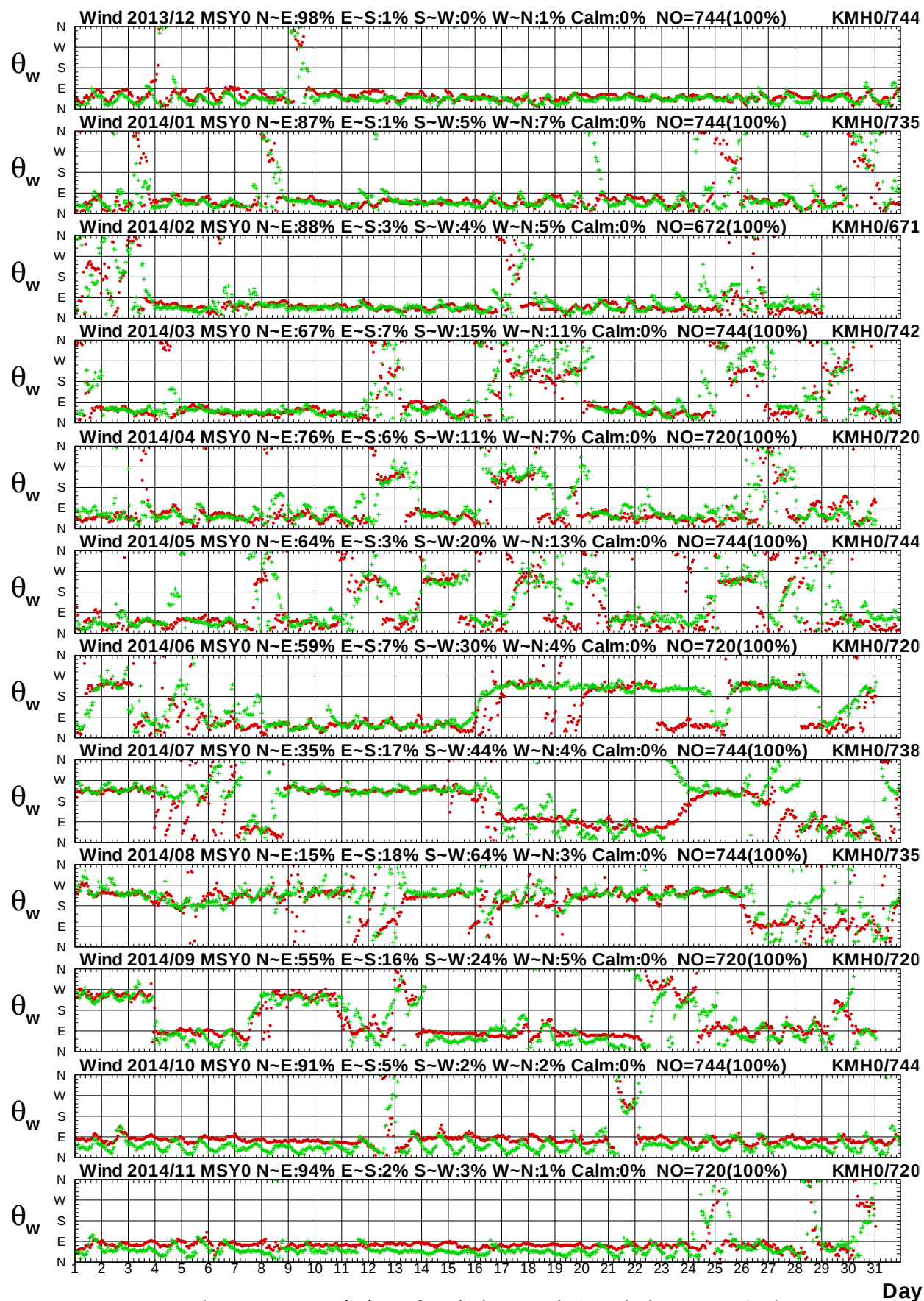
圖 1.10b 2014年每月馬祖海域 Y 站與金門海域 H 站風向圖
