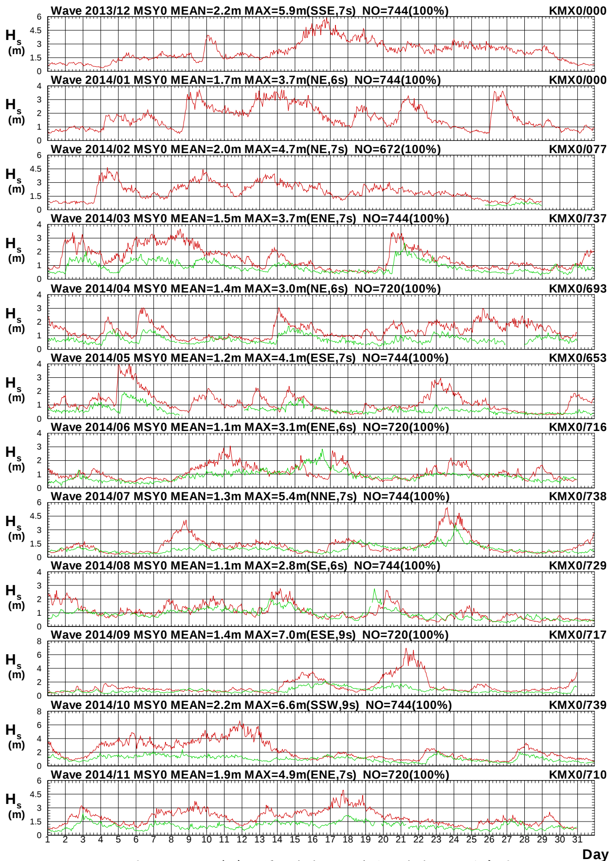
圖 2.3a 2014年每月馬祖海域 Y 站與金門海域 X 站波高圖
