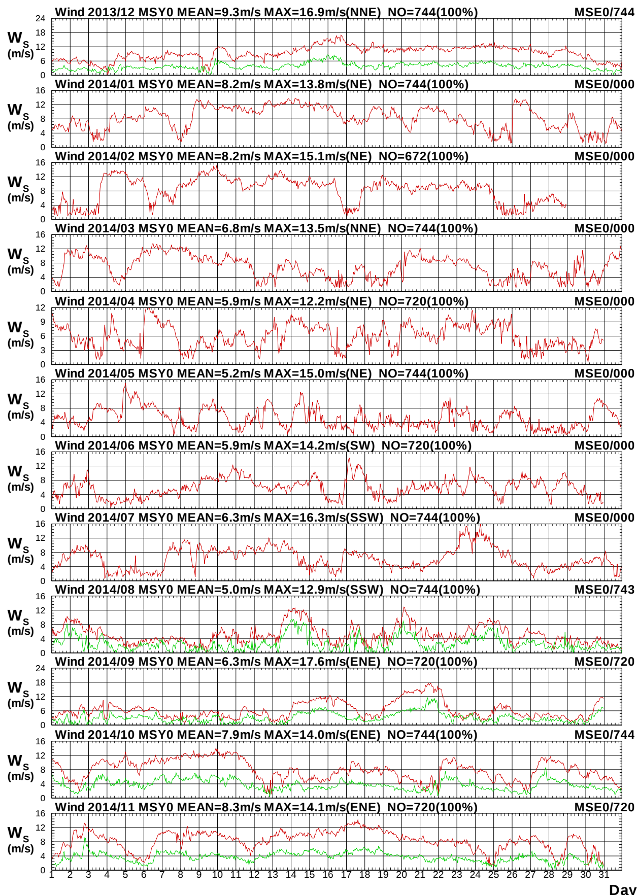
圖 1.3a 2014年每月馬祖海域 Y 站與 E 站風速比較圖
