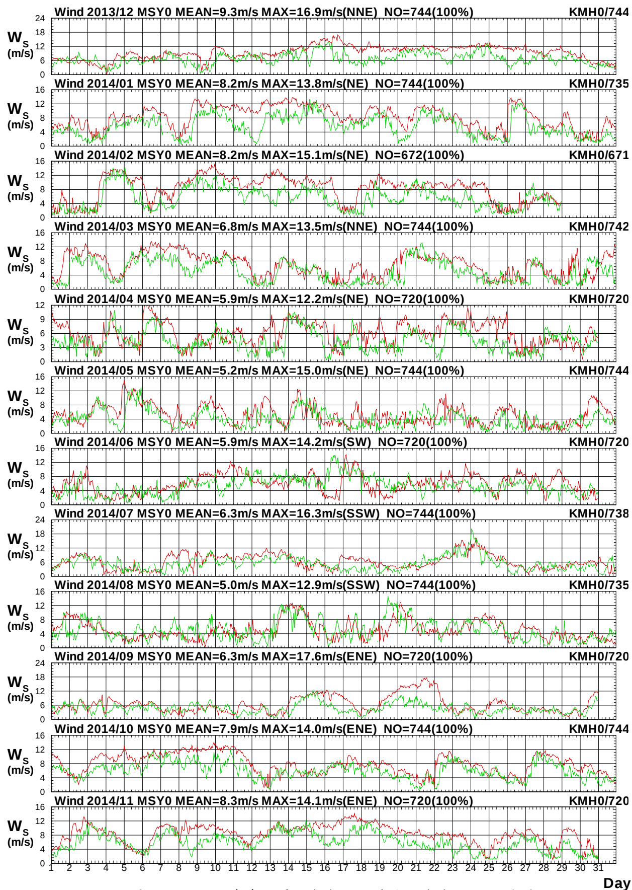
圖 1.10a 2014年每月馬祖海域 Y 站與金門海域 H 站風速圖
