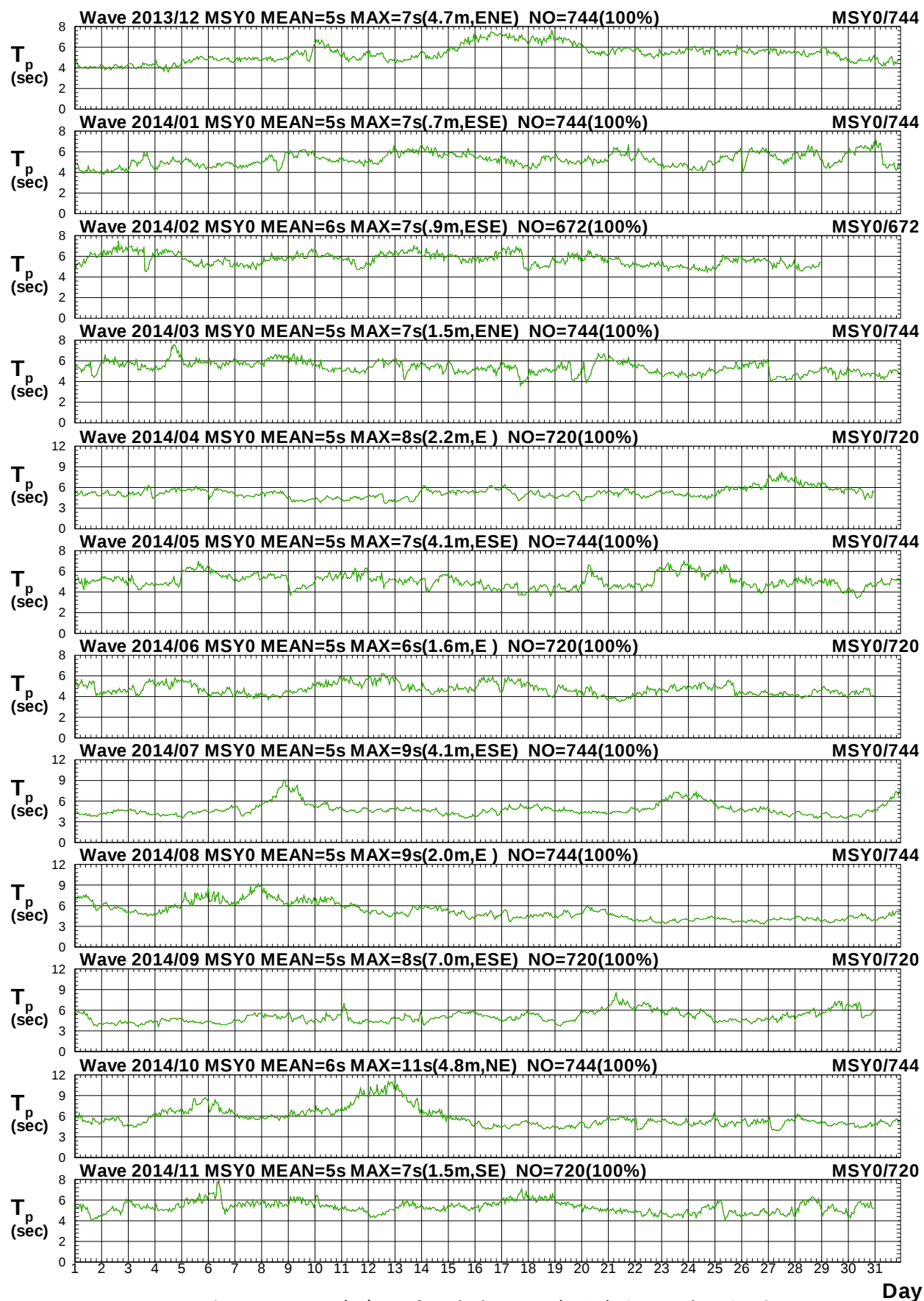
圖 2.1b 2014年每月馬祖海域 Y 站修補前後之週期比較圖
