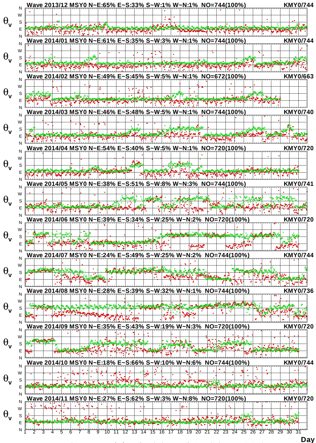
圖 2.4c 2014年每月馬祖海域 Y 站與金門海域 Y 站波向圖
