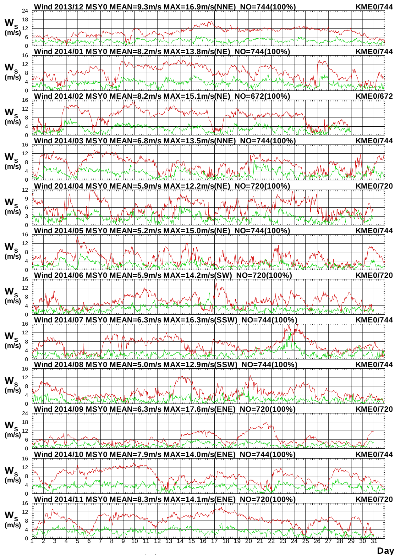
圖 1.9a 2014年每月馬祖海域 Y 站與金門海域 E 站風速圖
