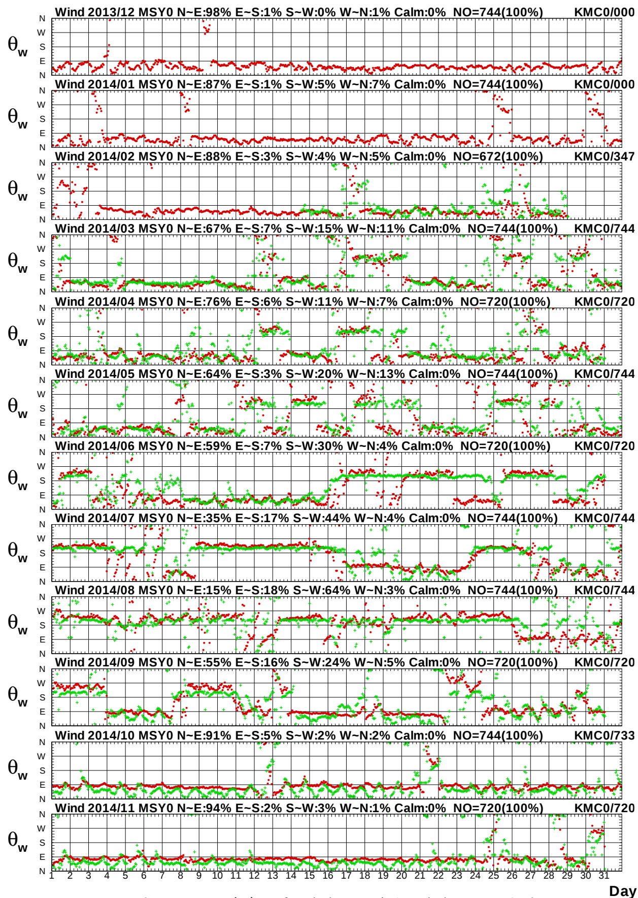
圖 1.7b 2014年每月馬祖海域 Y 站與金門海域 C 站風向圖
