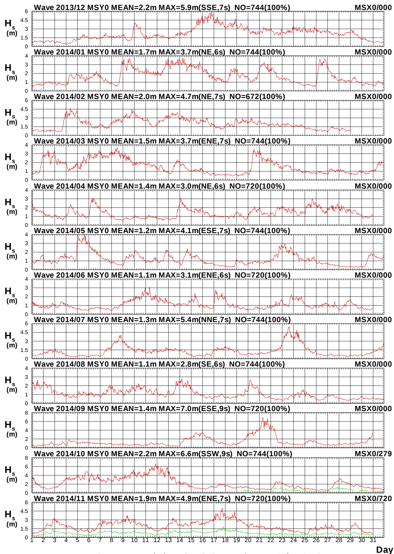
圖 2.2a 2014年每月馬祖海域 Y 站與 X 站波高比較圖
