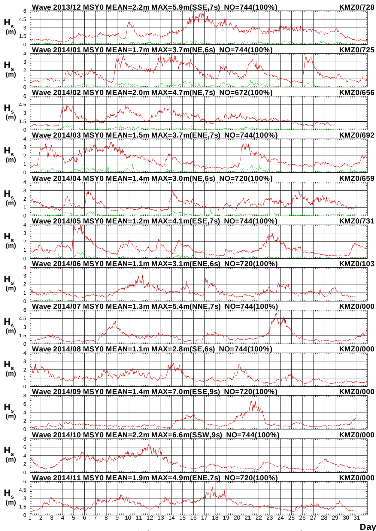
圖 2.5a 2014年每月馬祖海域 Y 站與金門海域 Z 站波高圖
