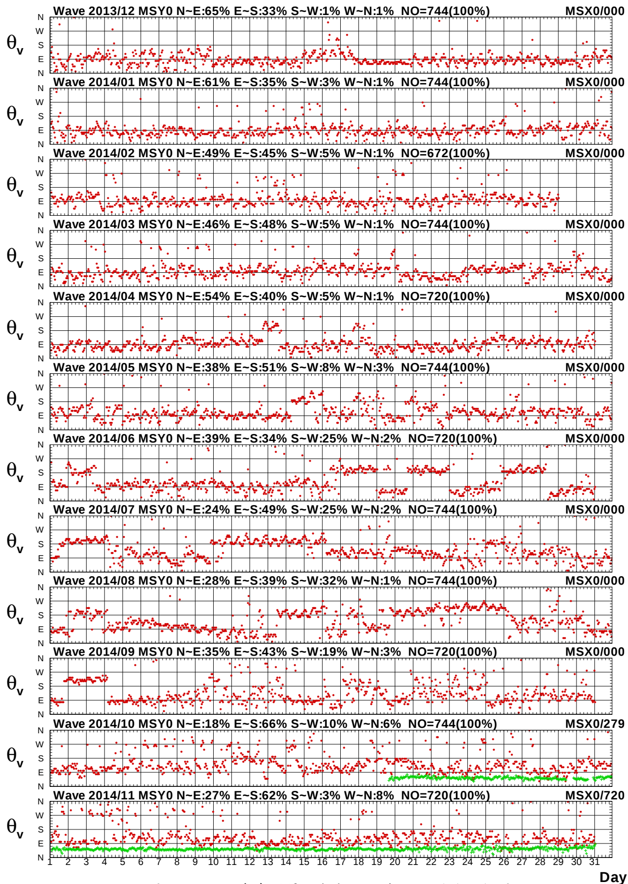
圖 2.2c 2014年每月馬祖海域 Y 站與 X 站波向比較圖
