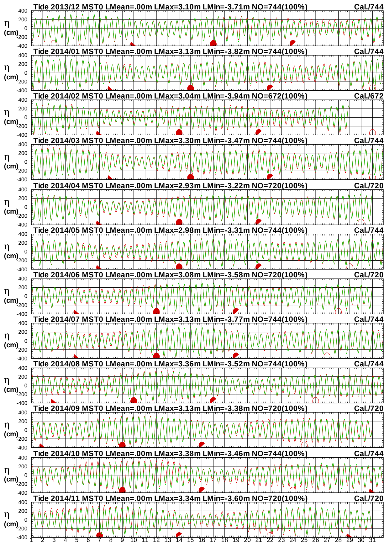
圖 3.1.2 2014 年每月馬祖海域 T 站潮位歷線圖 (綠線: 天文潮)
