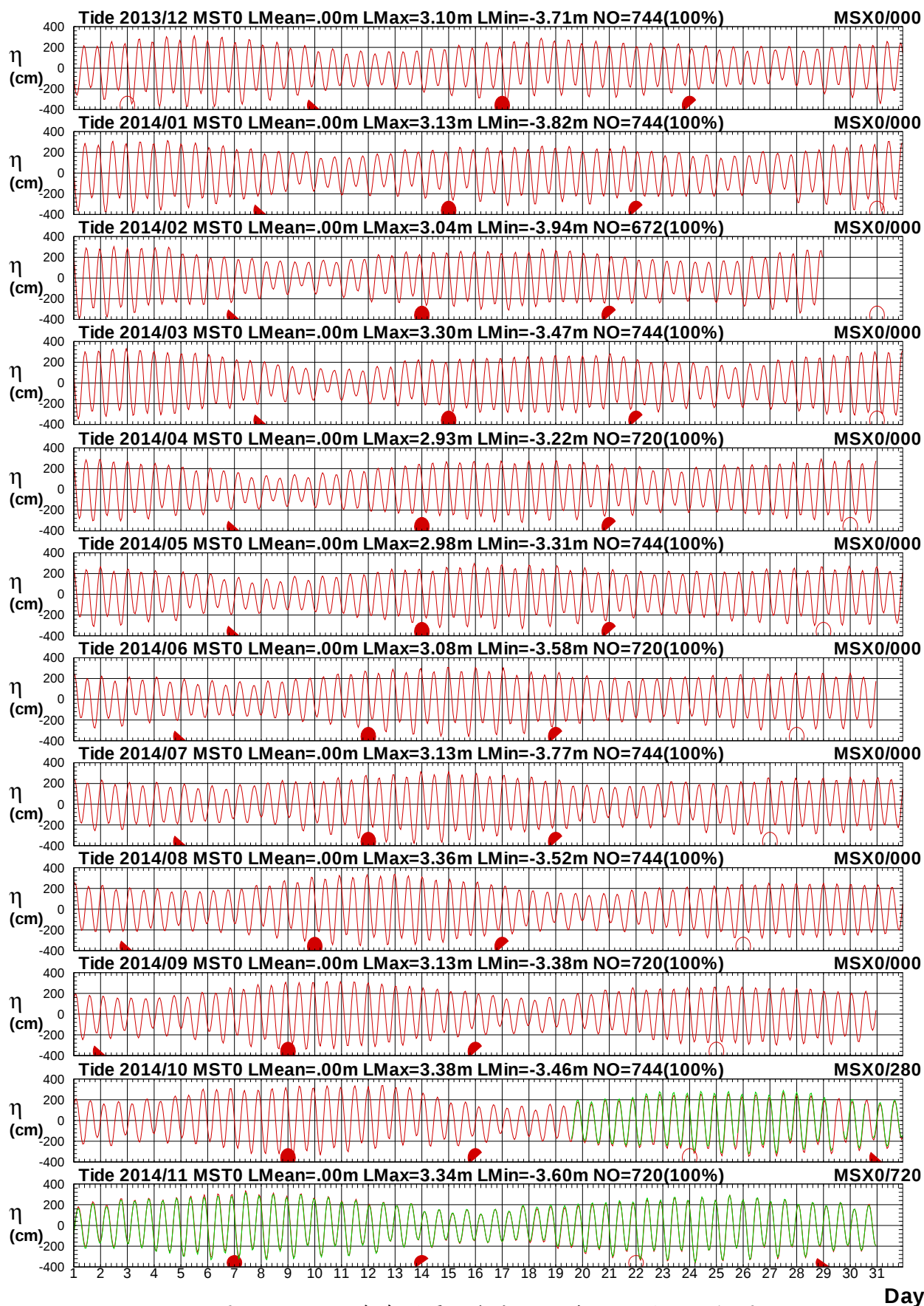
圖 3.1.4 2014 年每月馬祖海域 T 站與 X 站潮位比較圖
