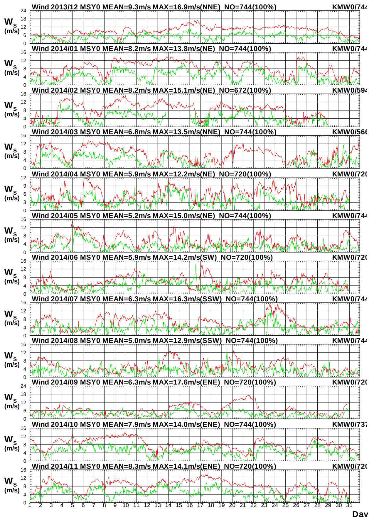
圖 1.5a 2014年每月馬祖海域 Y 站與金門海域 W 站風速圖
