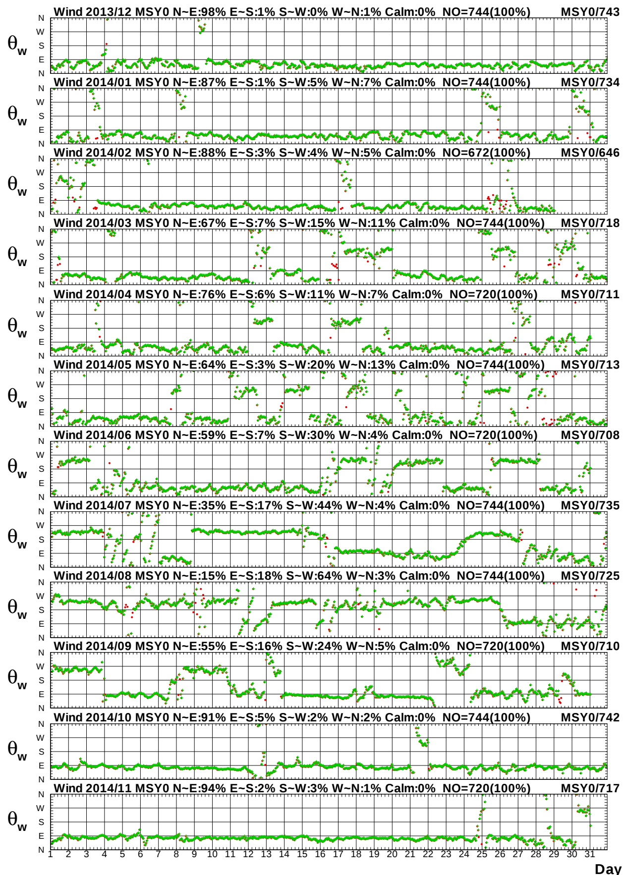
圖 1.1b 2014年每月馬祖海域 Y 站修補前後之風向比較圖
