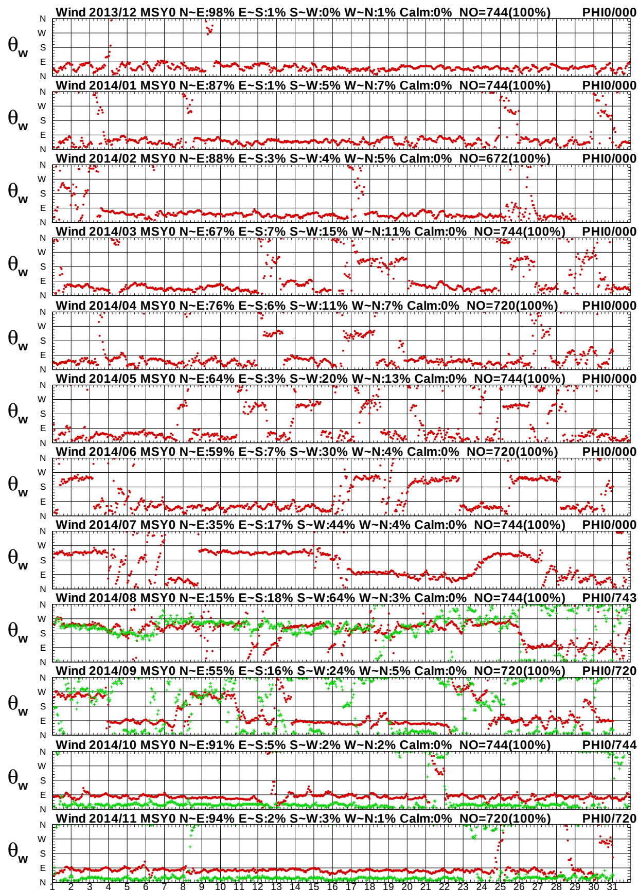
圖 1.17b 2014年每月馬祖海域 Y 站與澎湖海域 I 站風向圖
