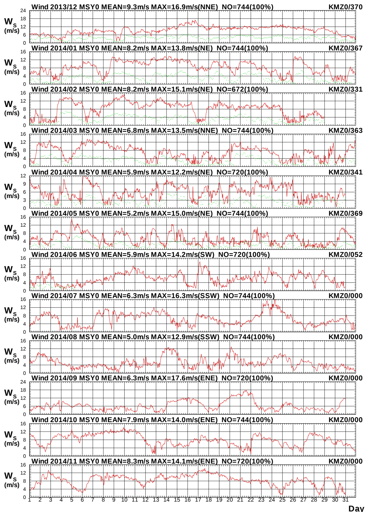
圖 1.8a 2014年每月馬祖海域 Y 站與金門海域 Z 站風速圖
