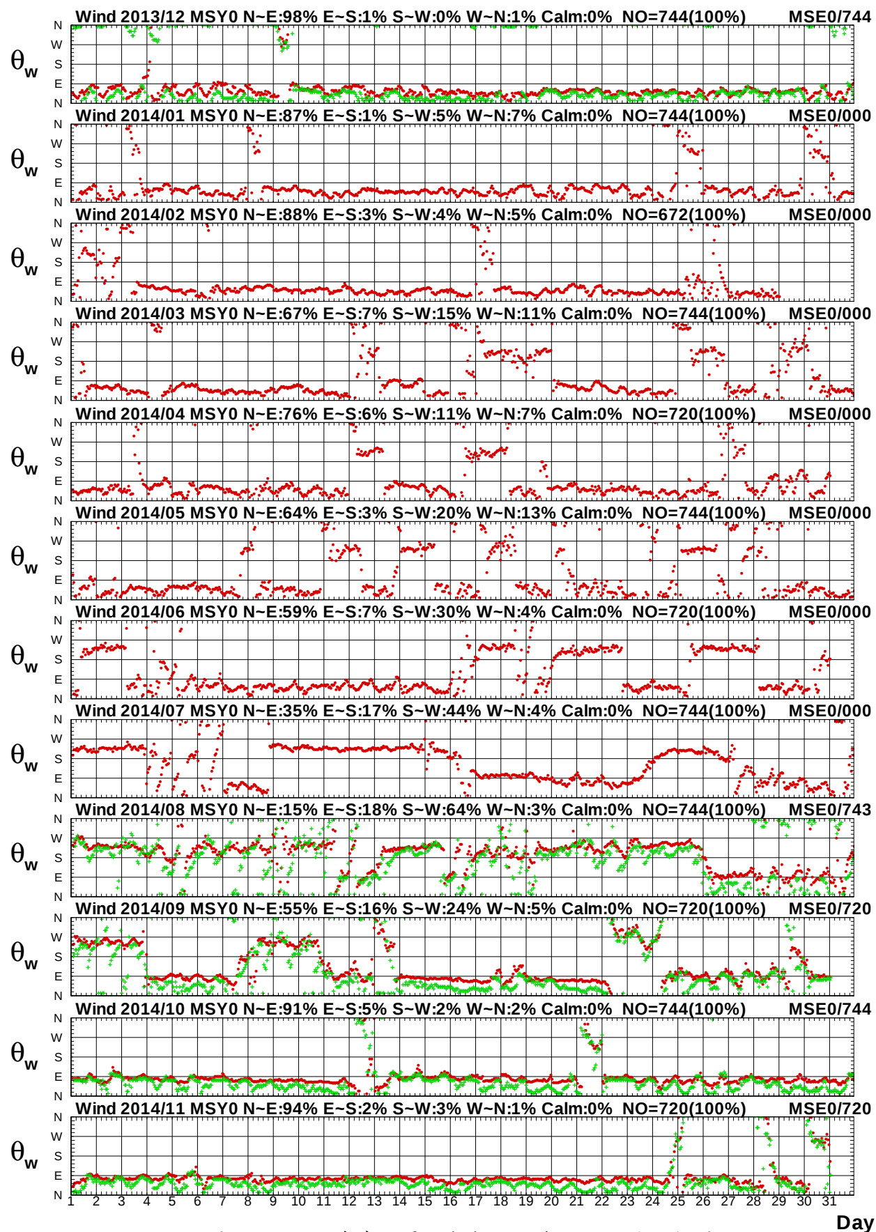
圖 1.3b 2014年每月馬祖海域 Y 站與 E 站風向比較圖
