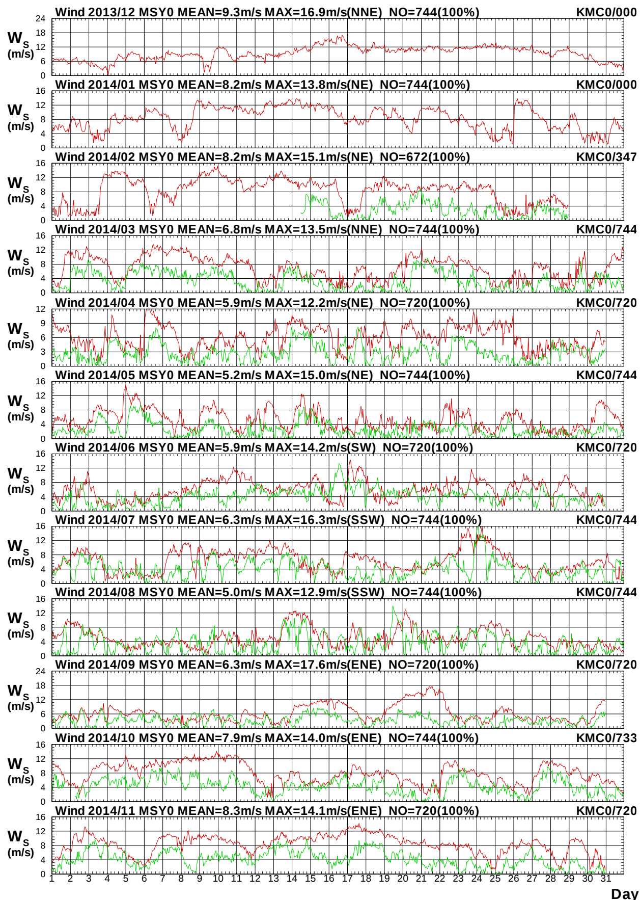
圖 1.7a 2014年每月馬祖海域 Y 站與金門海域 C 站風速圖
