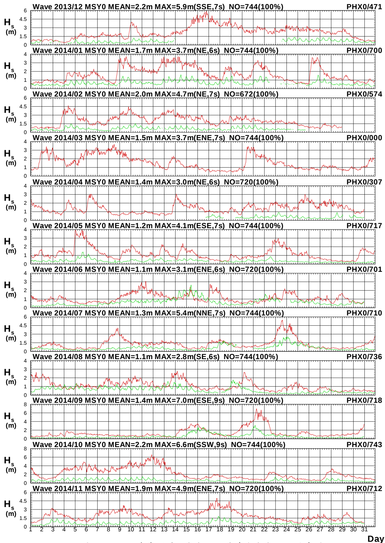
圖 2.7a 2014年每月馬祖海域 Y 站與澎湖海域 X 站波高圖
