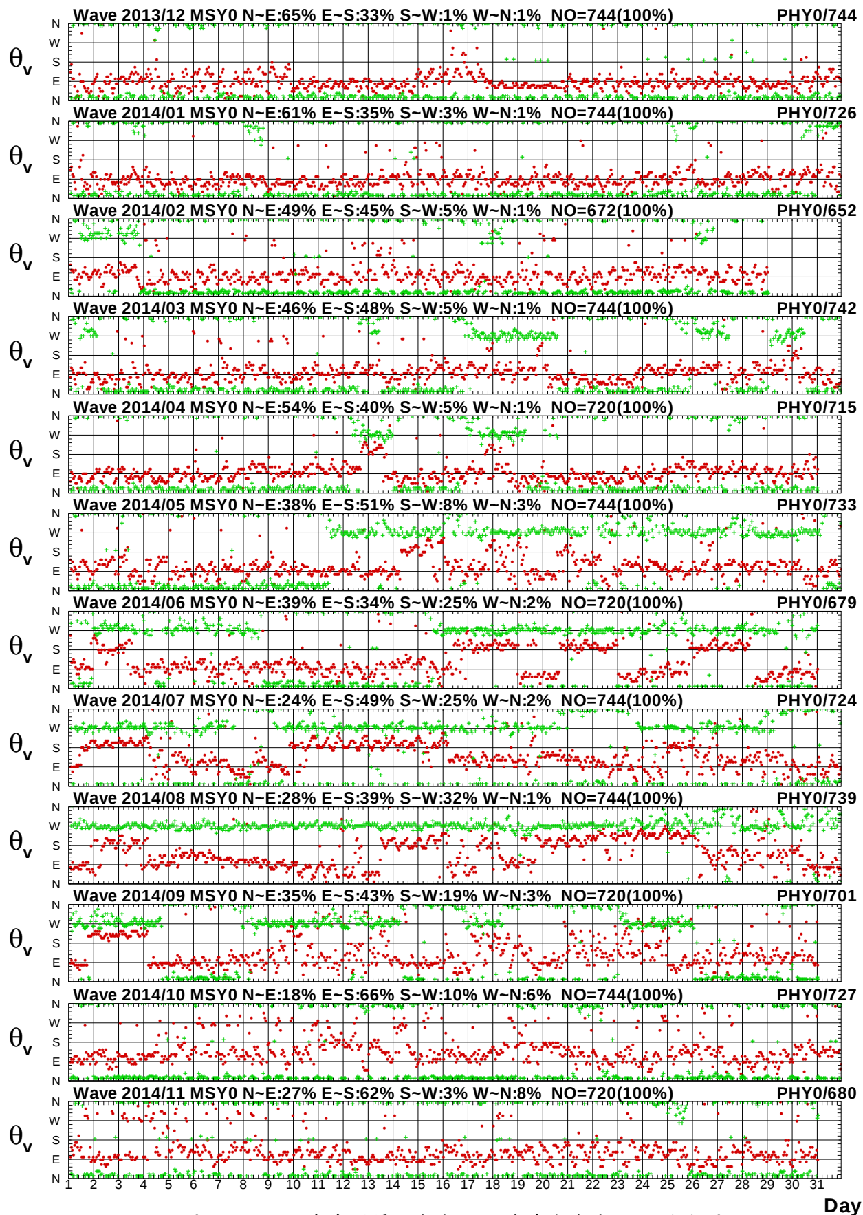
圖 2.8c 2014 年每月馬祖海域 Y 站與澎湖海域 Y 站波向圖
