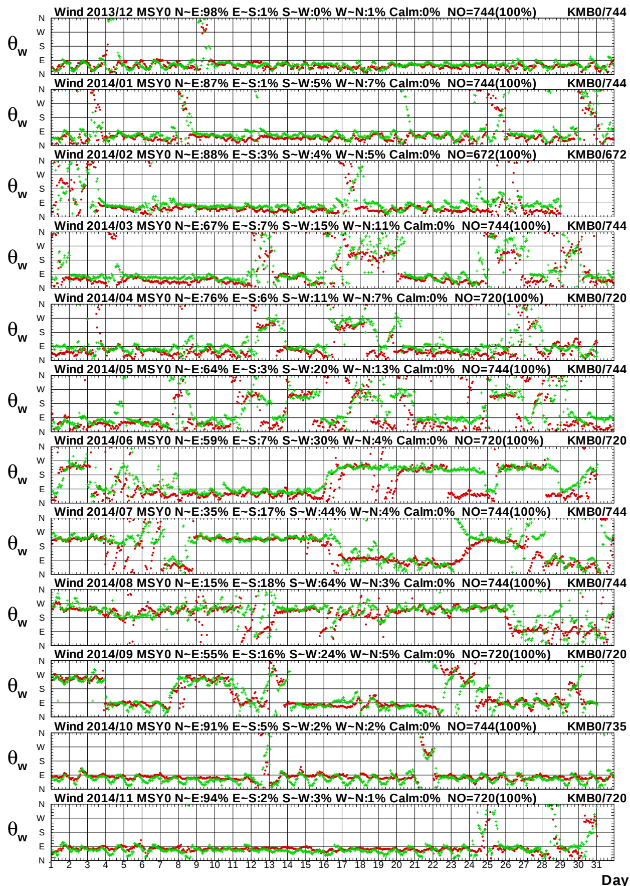
圖 1.6b 2014年每月馬祖海域 Y 站與金門海域 B 站風向圖
