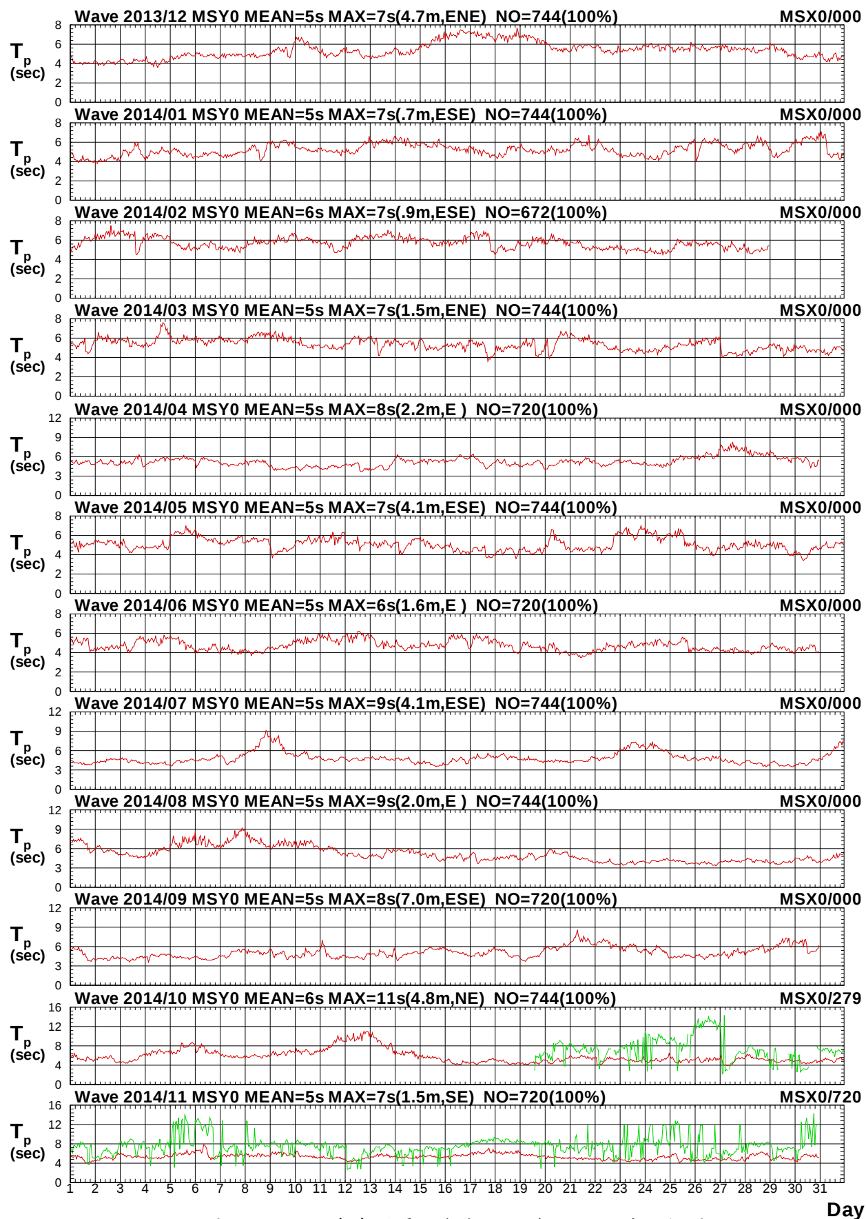
圖 2.2b 2014 年每月馬祖海域 Y 站與 X 站週期比較圖
