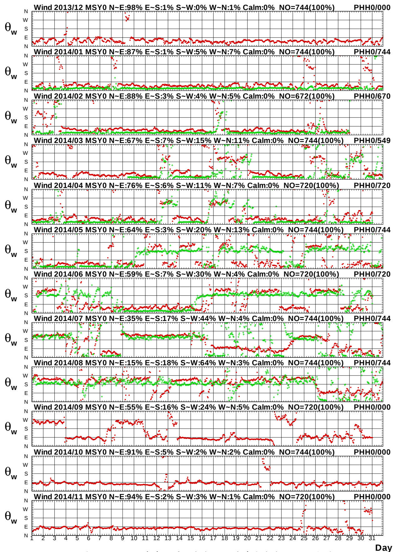
圖 1.16b 2014年每月馬祖海域 Y 站與澎湖海域 H 站風向圖
