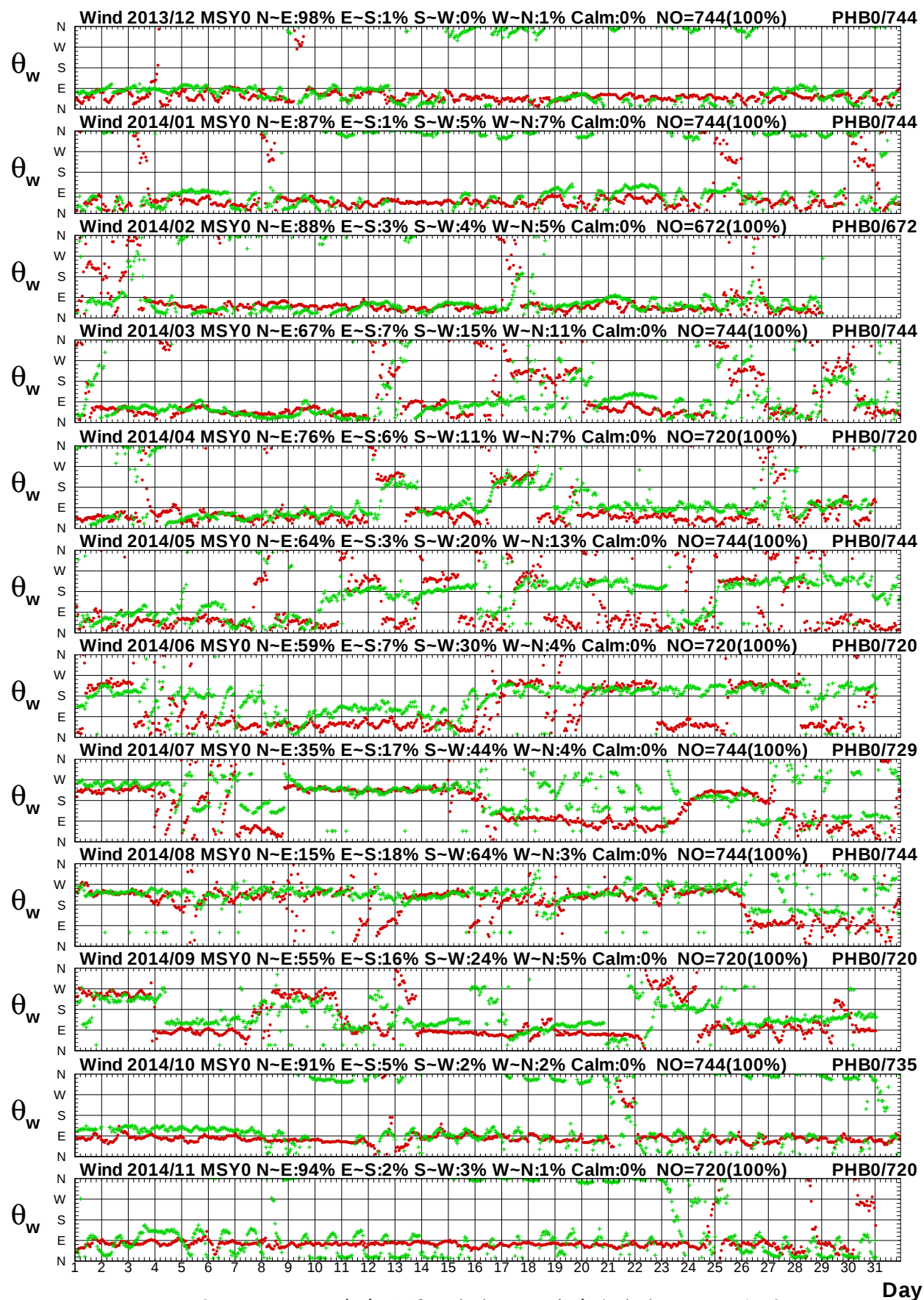
圖 1.14b 2014年每月馬祖海域 Y 站與澎湖海域 B 站風向圖
