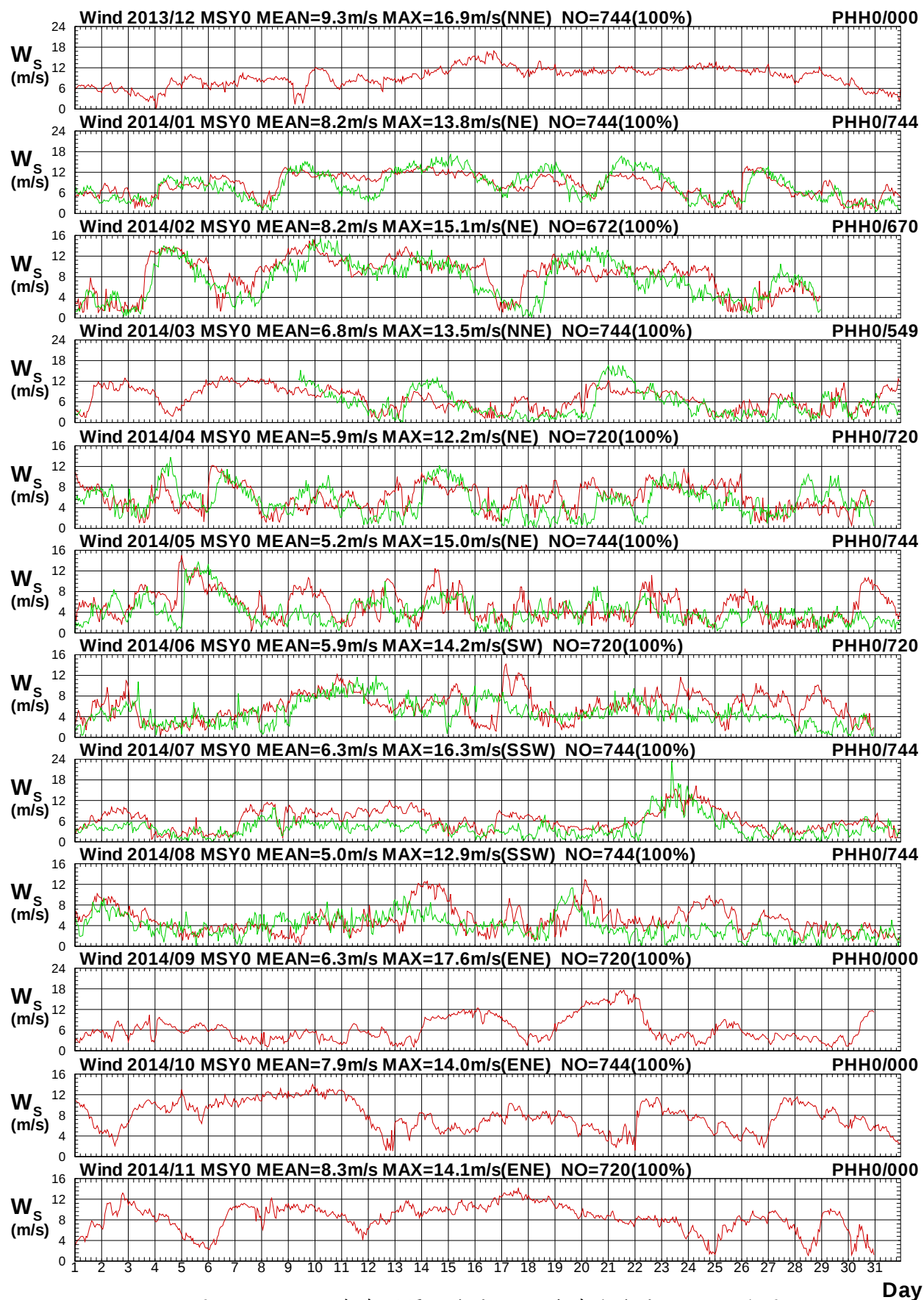
圖 1.16a 2014年每月馬祖海域 Y 站與澎湖海域 H 站風速圖
