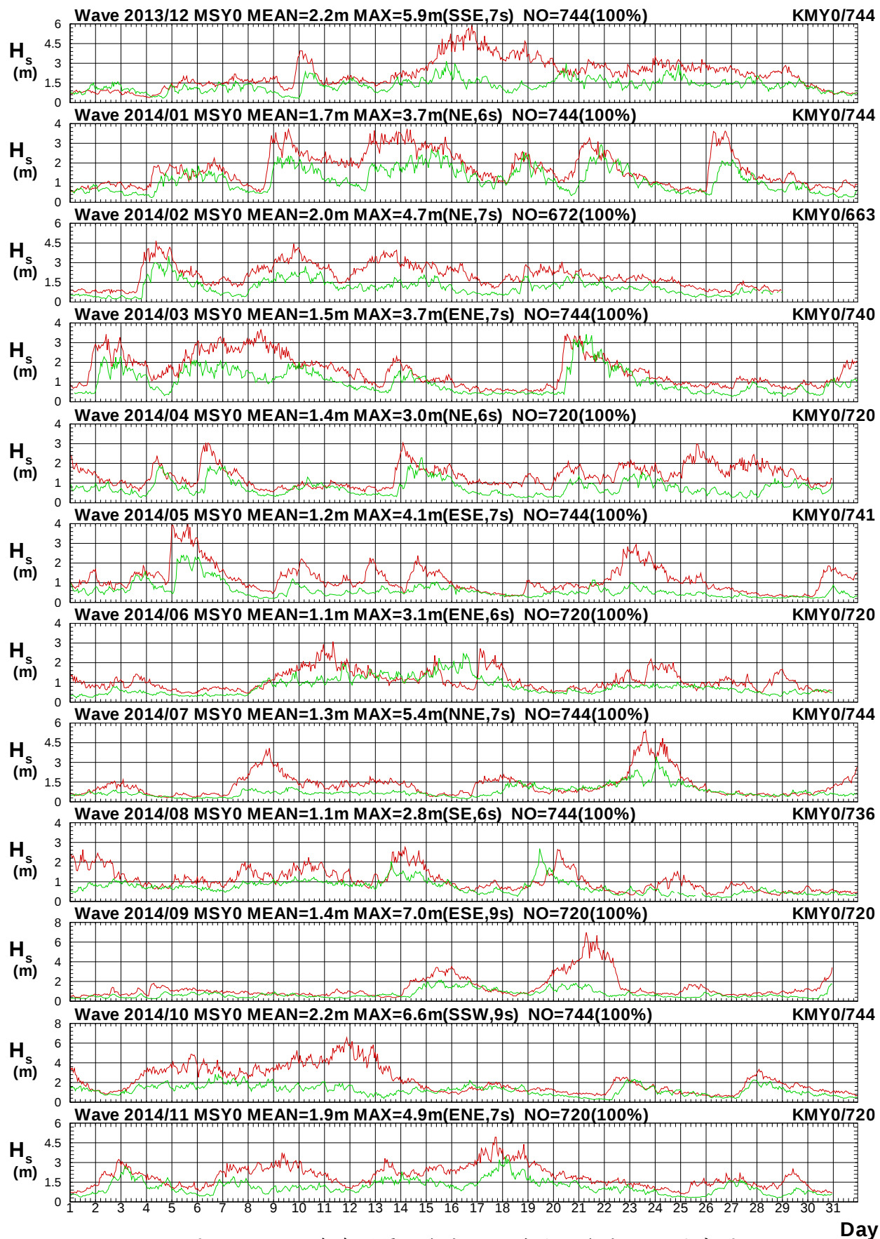
圖 2.4a 2014年每月馬祖海域 Y 站與金門海域 Y 站波高圖
