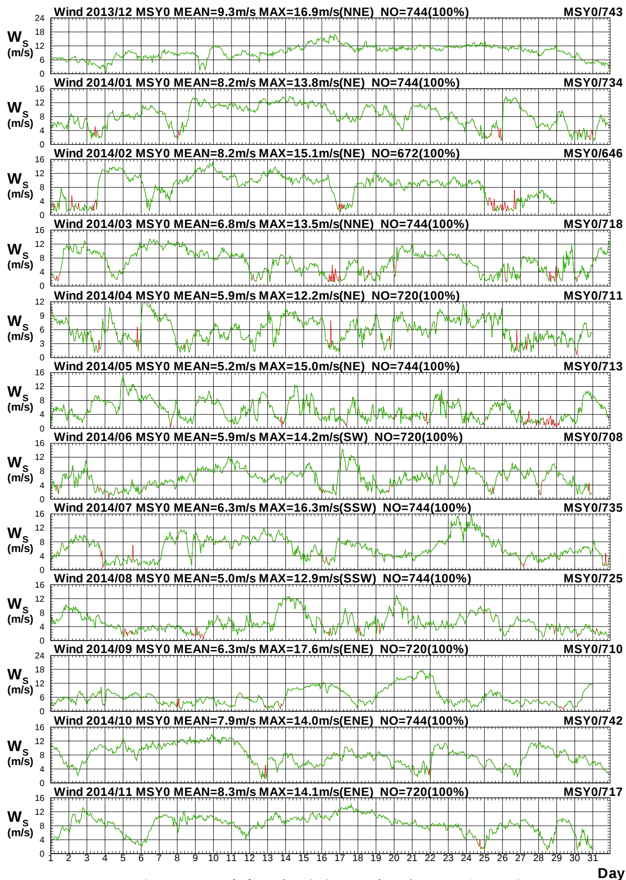
圖 1.1a 2014年每月馬祖海域 Y 站修補前後之風速比較圖
