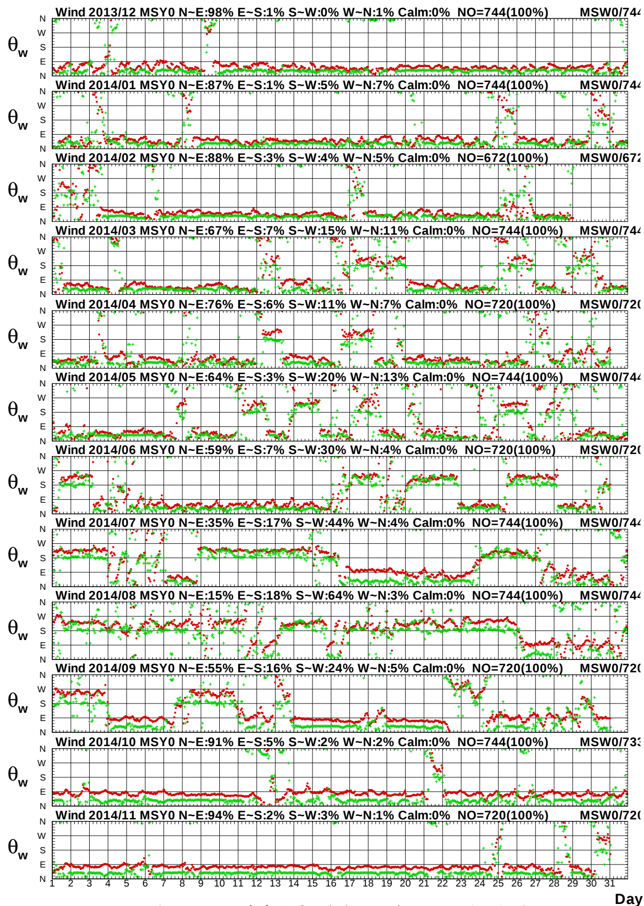
圖 1.2b 2014 年每月馬祖海域 Y 站與 W 站風向比較圖
