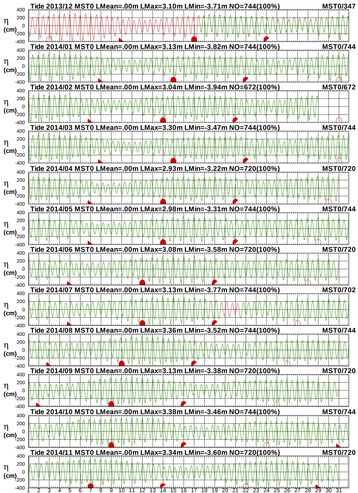
圖 3.1.1 2014 年每月馬祖海域 T 站修補前後之潮位比較圖
