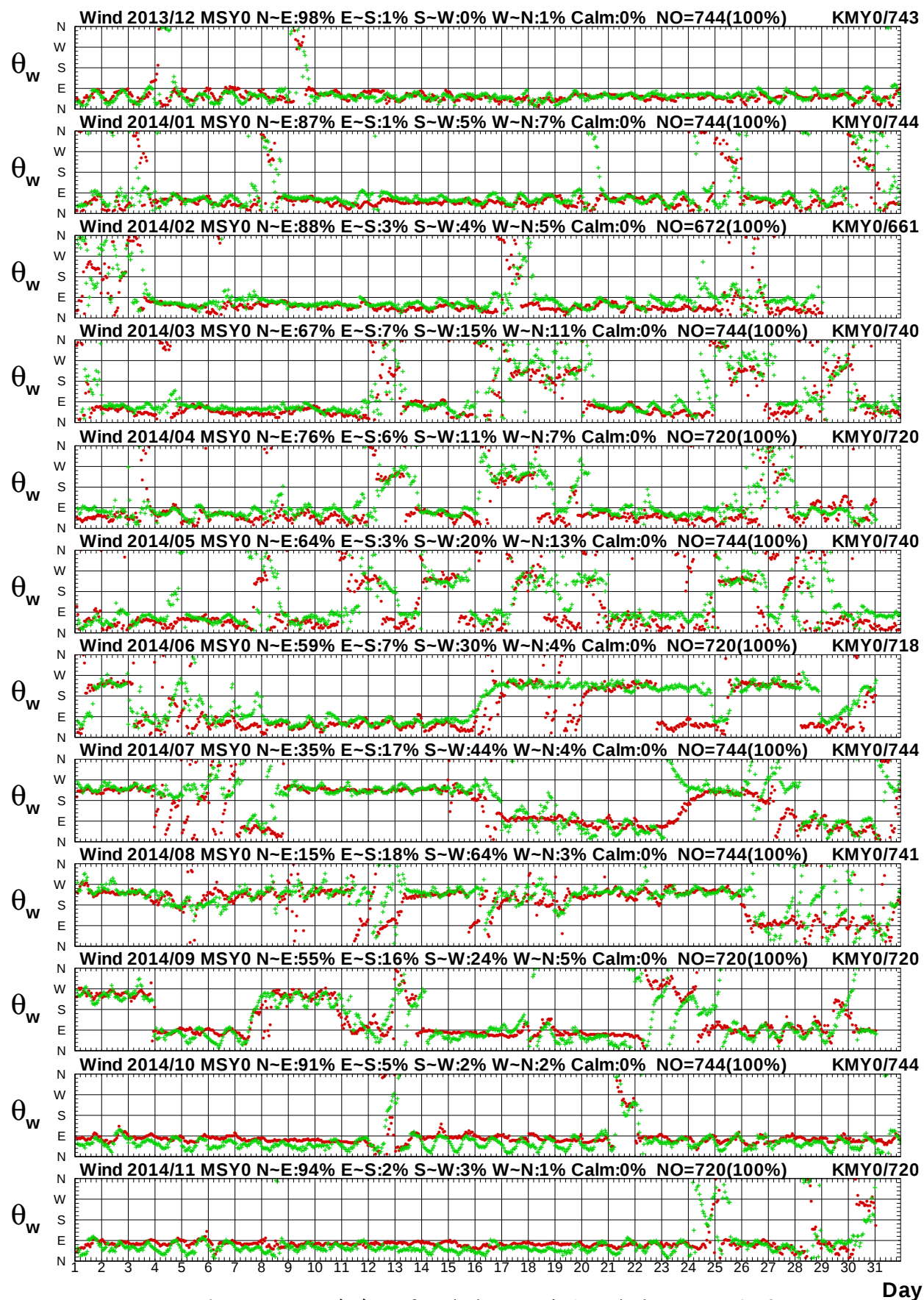
圖 1.4b 2014年每月馬祖海域 Y 站與金門海域 Y 站風向圖
