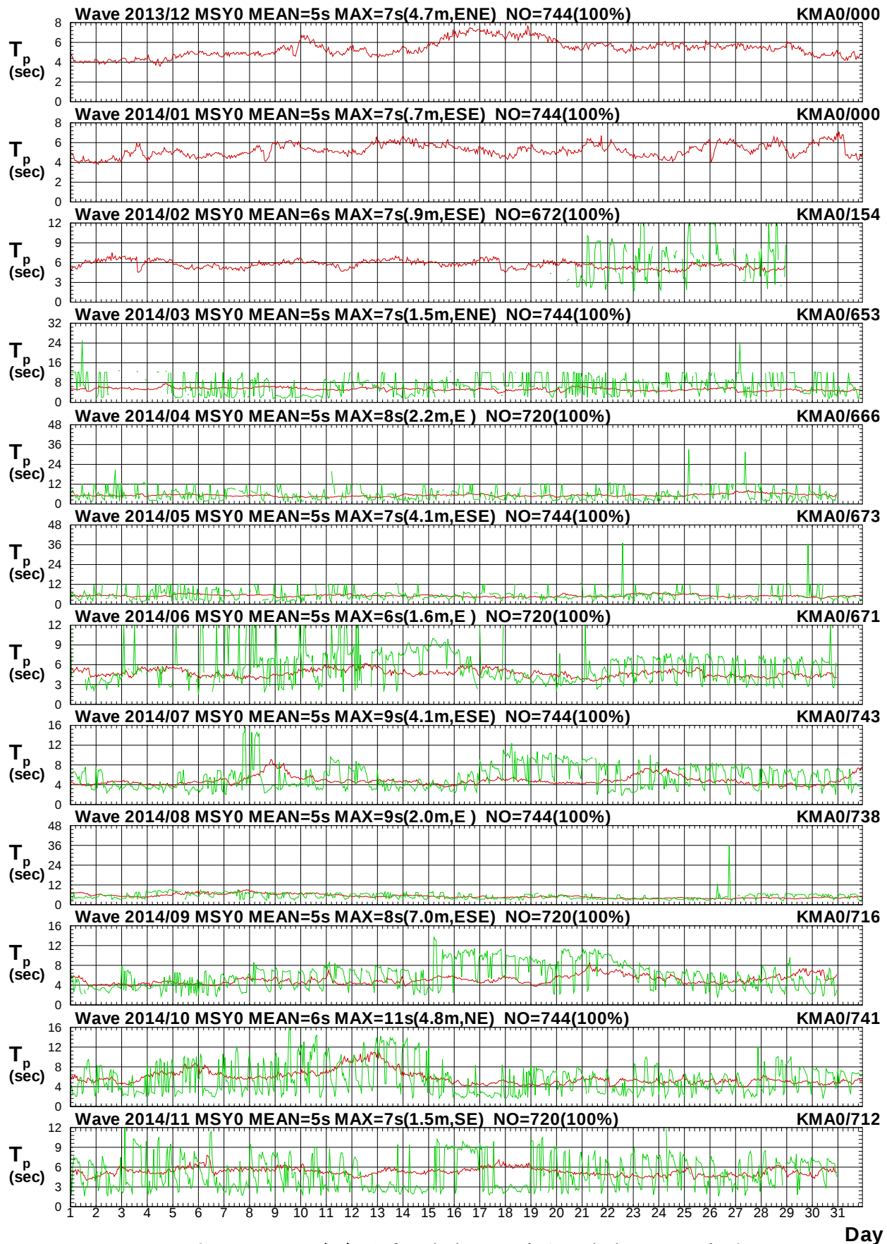
圖 2.6b 2014年每月馬祖海域 Y 站與金門海域 A 站週期圖
