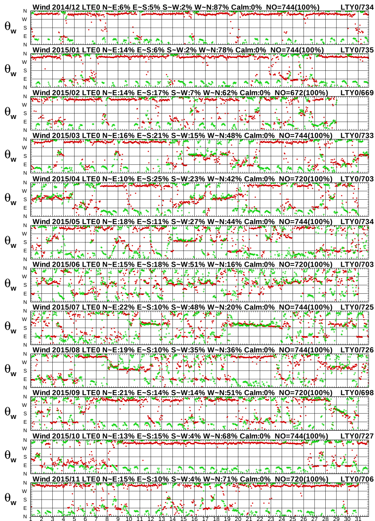
圖 1.5b 2015年每月臺東海域 E 站與 Y 站風向比較圖
