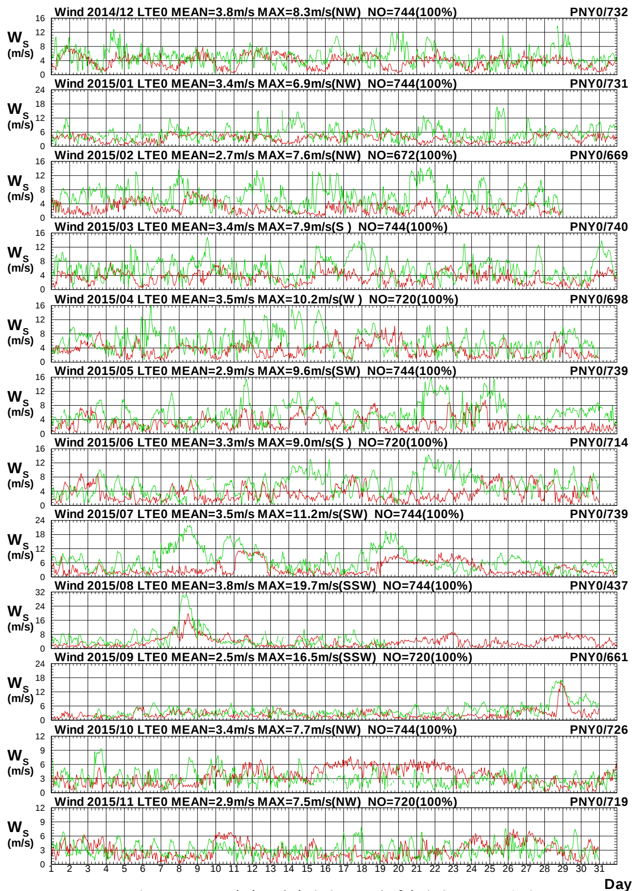
圖 1.16a 2015 年每月臺東海域 E 站與屏東海域 Y 站風速圖
