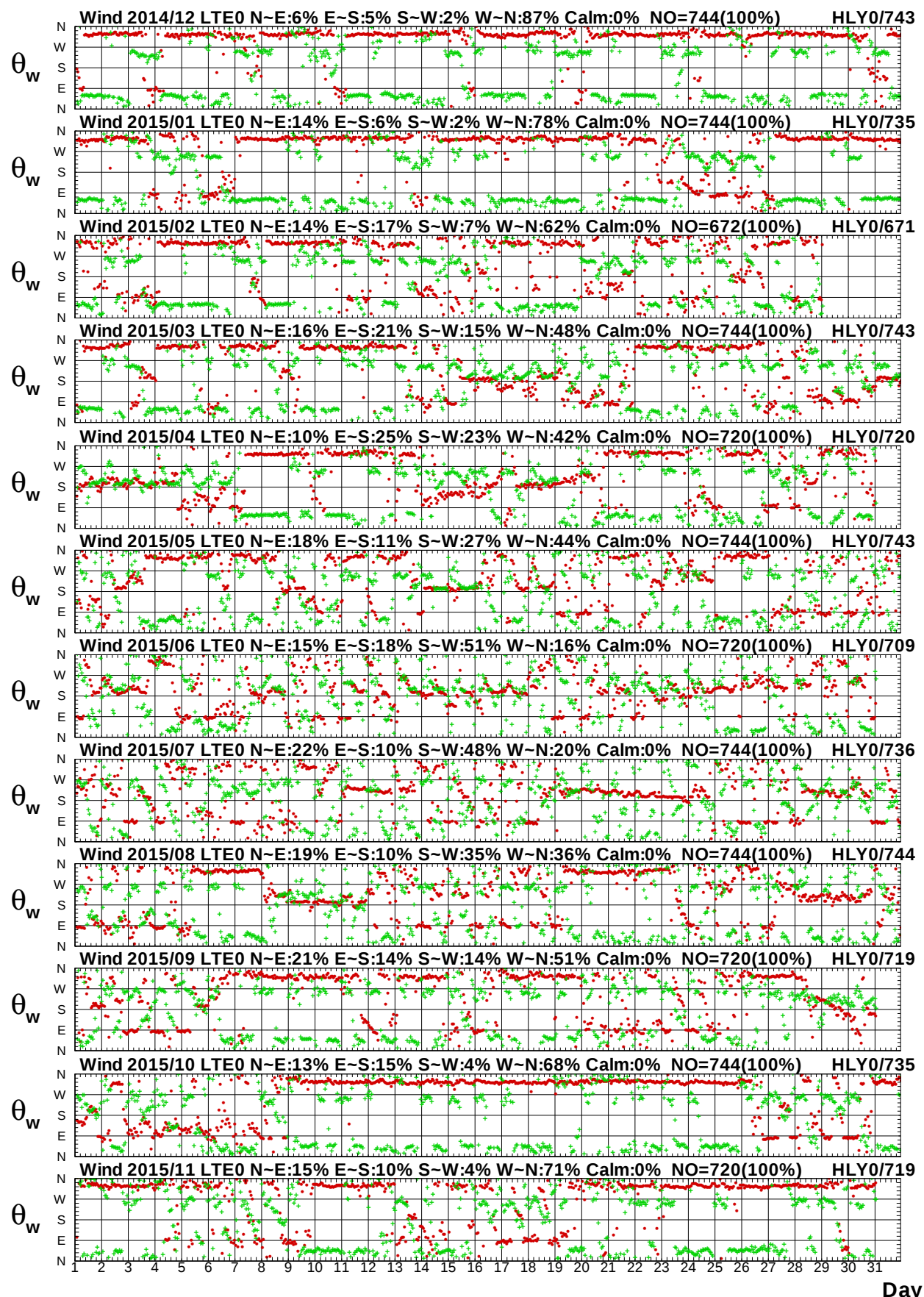
圖 1.12b 2015年每月臺東海域 E 站與花蓮海域 Y 站風向圖
