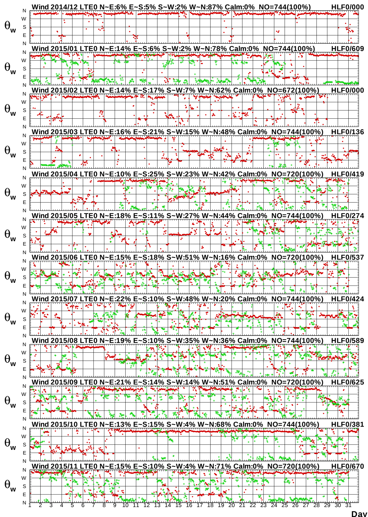
圖 1.15b 2015年每月臺東海域 E 站與花蓮海域 F 站風向圖
