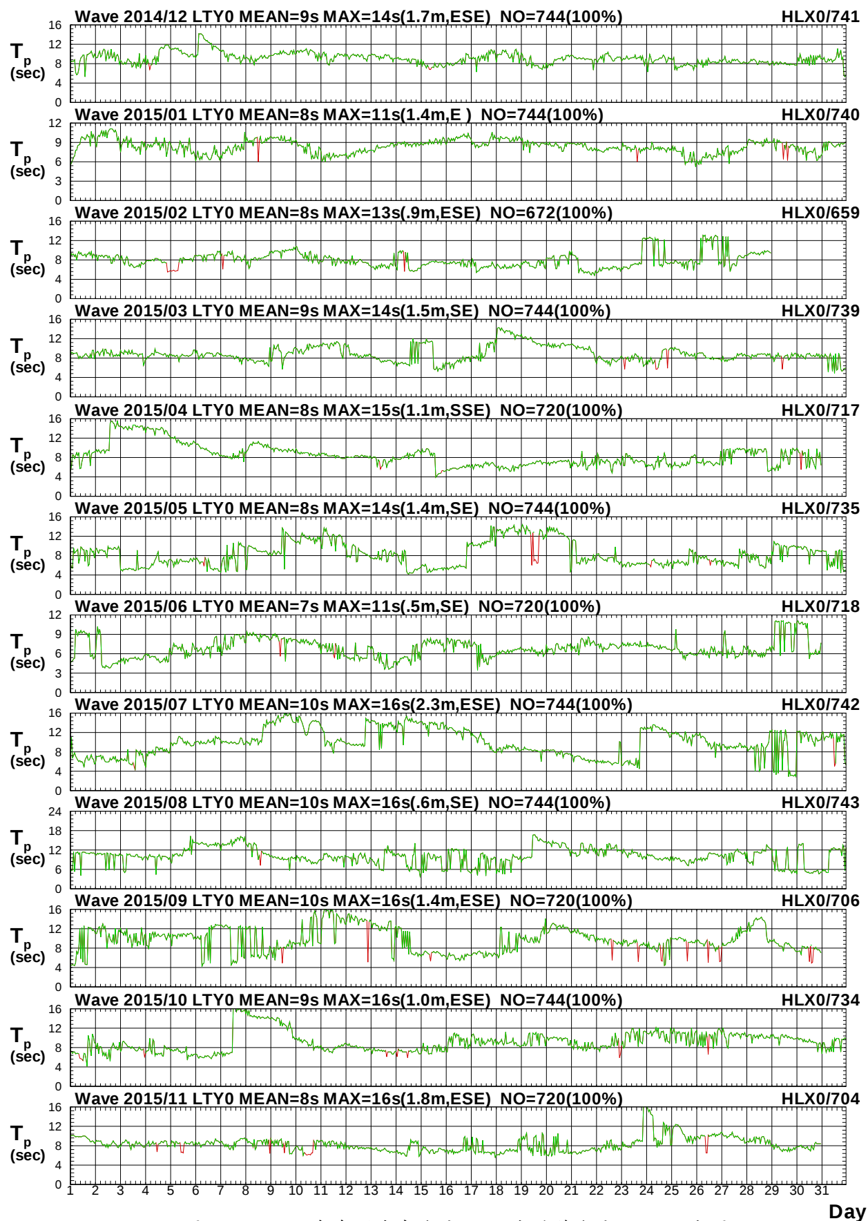
圖 2.3b 2015年每月臺東海域 Y 站與花蓮海域 X 站週期圖
