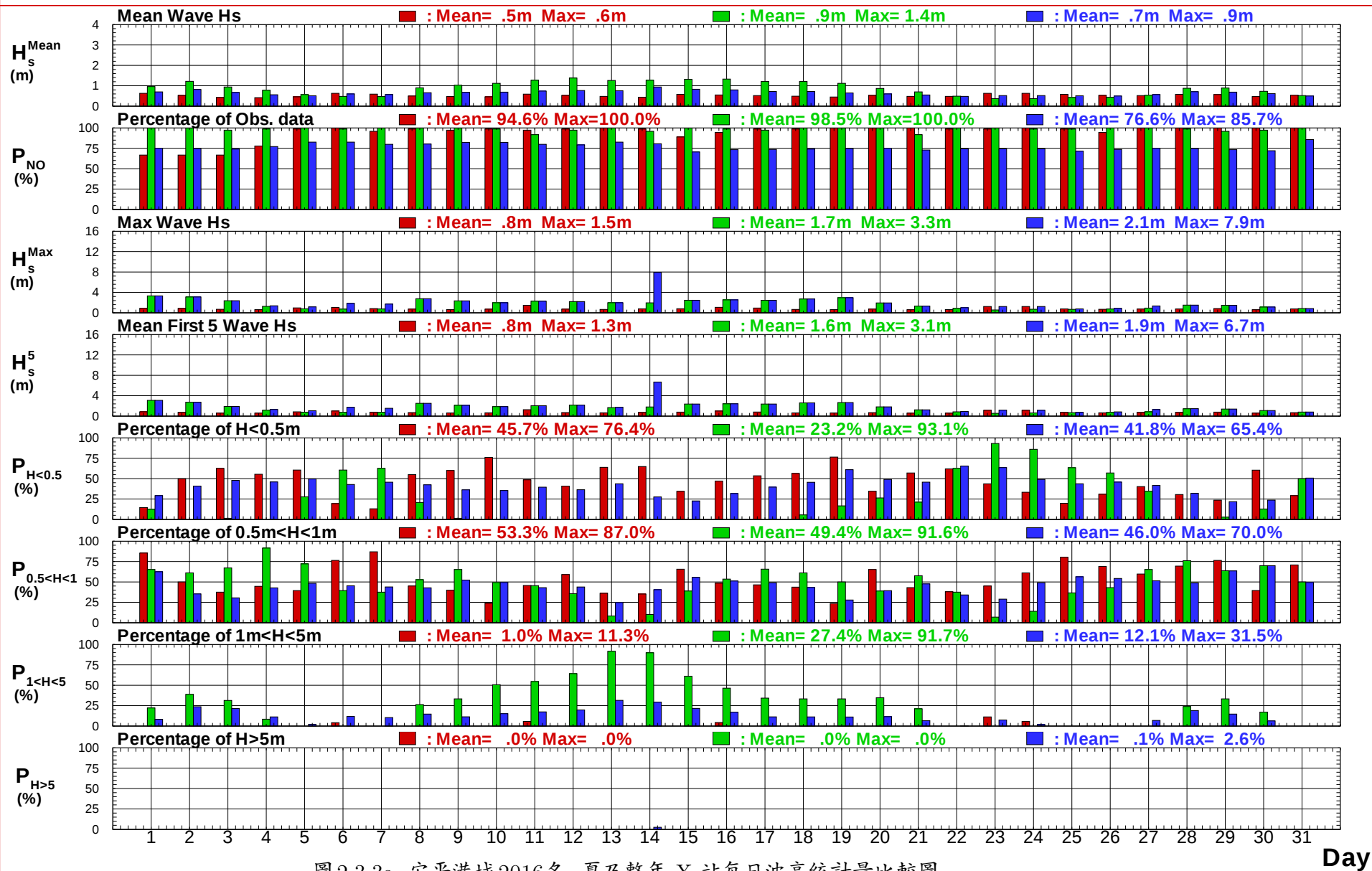
圖 2.3.3a 安平港域2016冬, 夏及整年 X 站每日波高統計量比較圖
