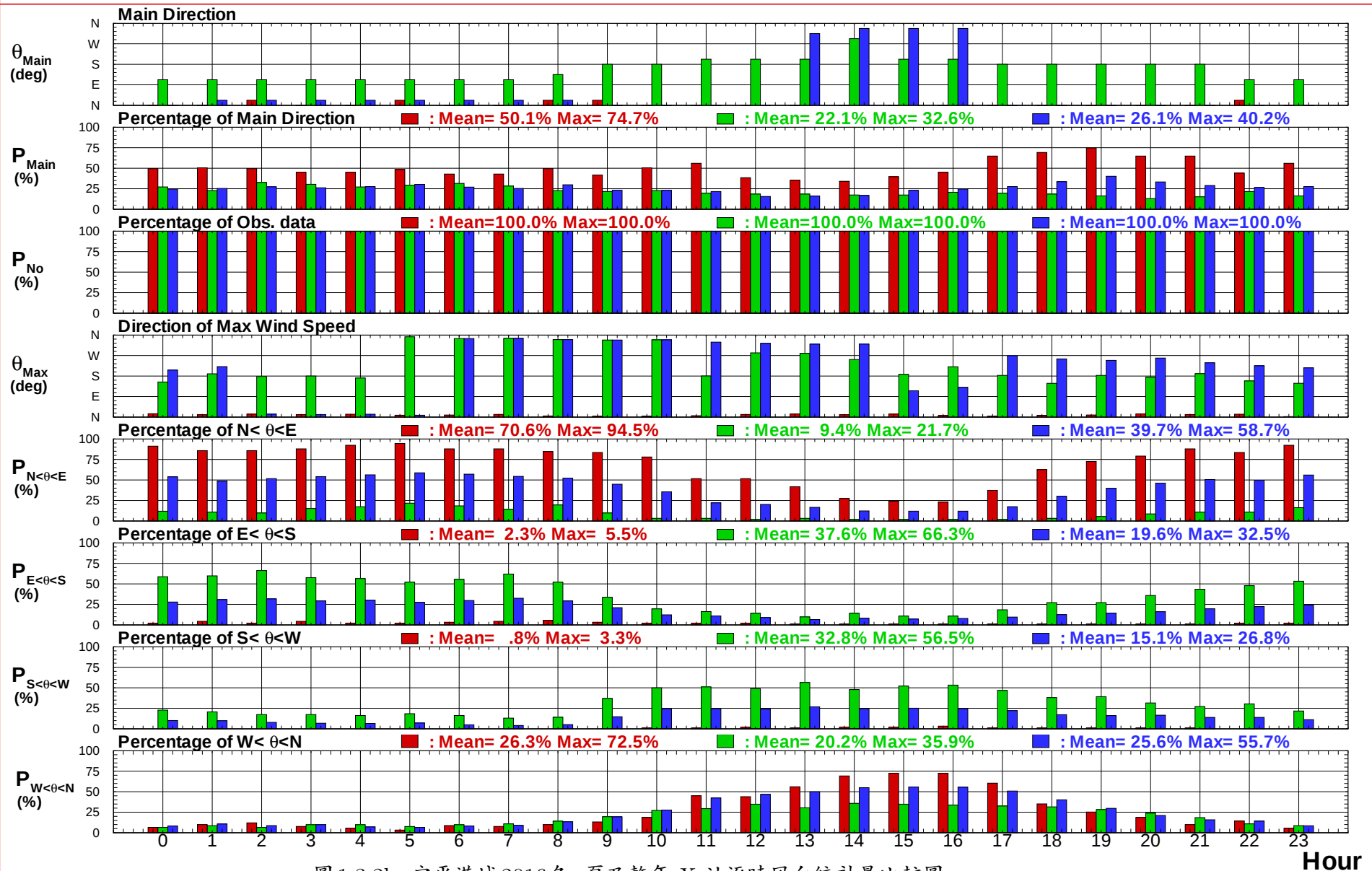
圖 1.3.2b 安平港域2016冬, 夏及整年 X 站逐時風向統計量比較圖
