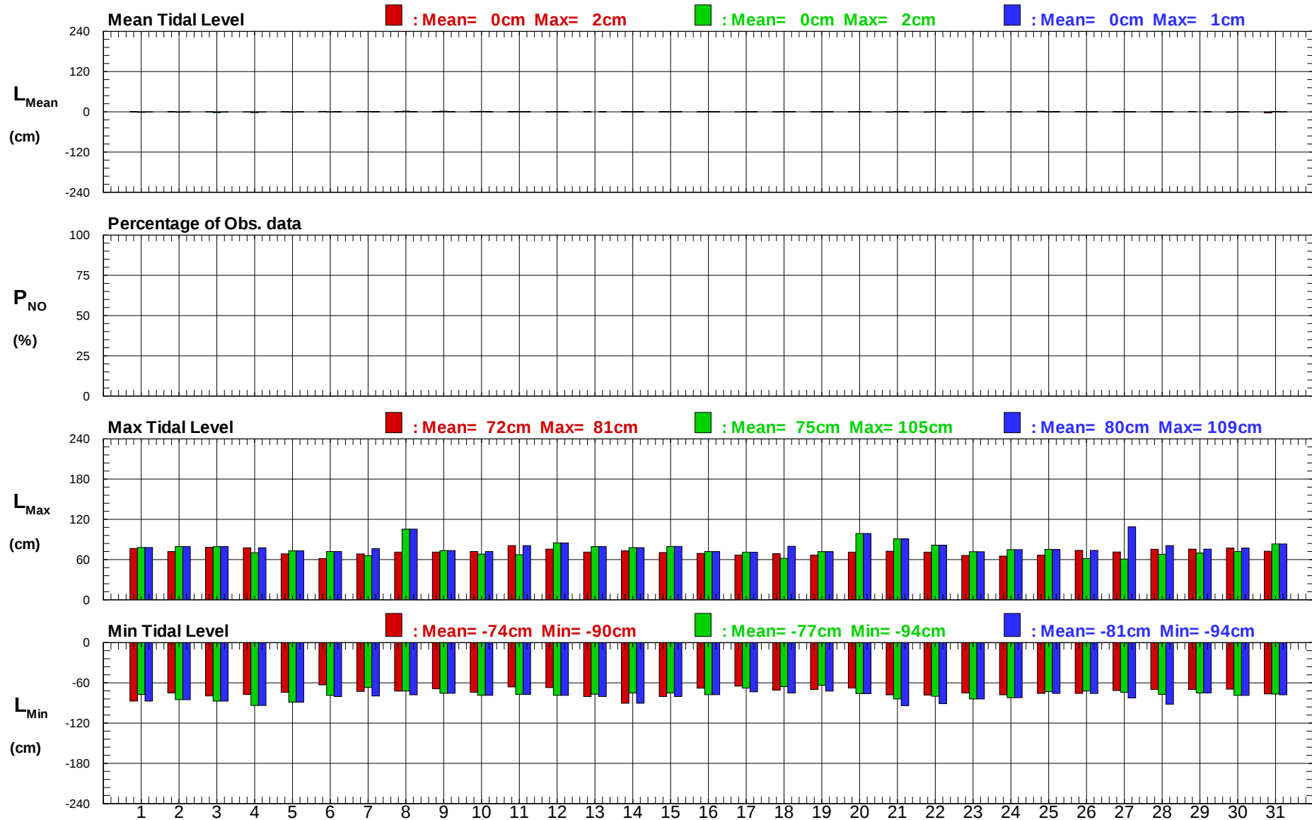
圖3.3.3b 安平港域歷年冬, 夏及整年 T 站每日潮位統計量比較圖
