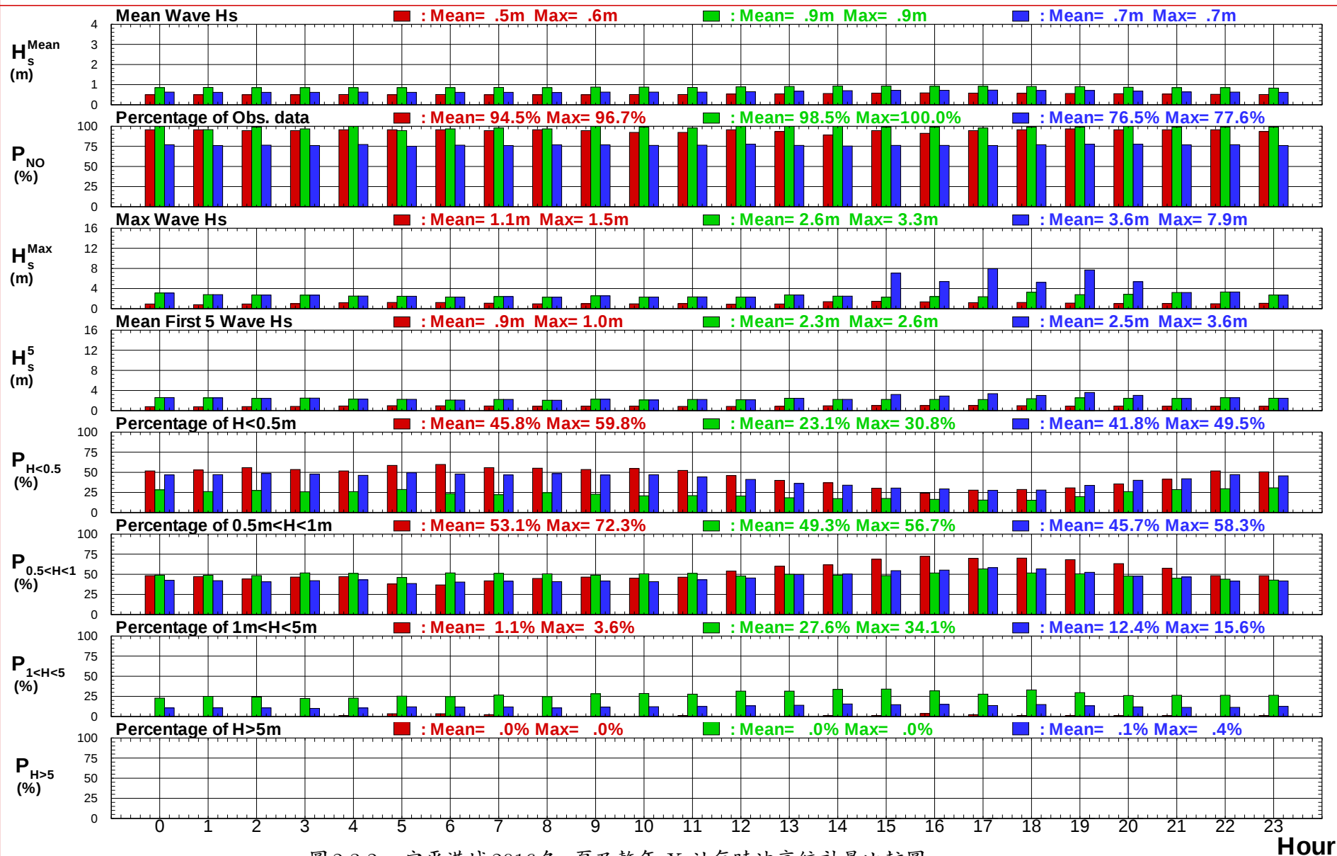
圖 2.3.2a 安平港域2016冬, 夏及整年 X 站每時波高統計量比較圖
