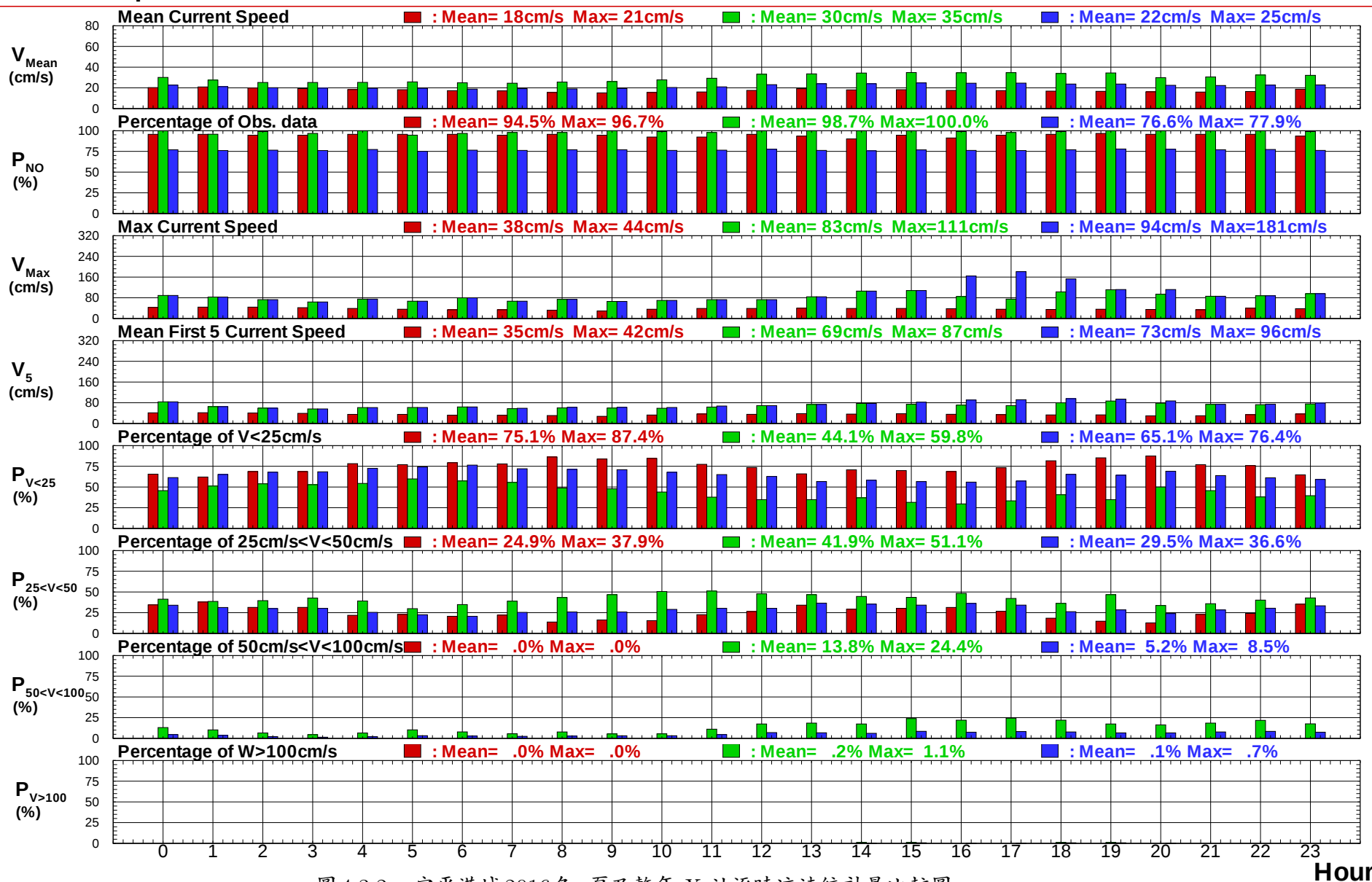
圖 4.3.2a 安平港域2016冬, 夏及整年 X 站逐時流速統計量比較圖
