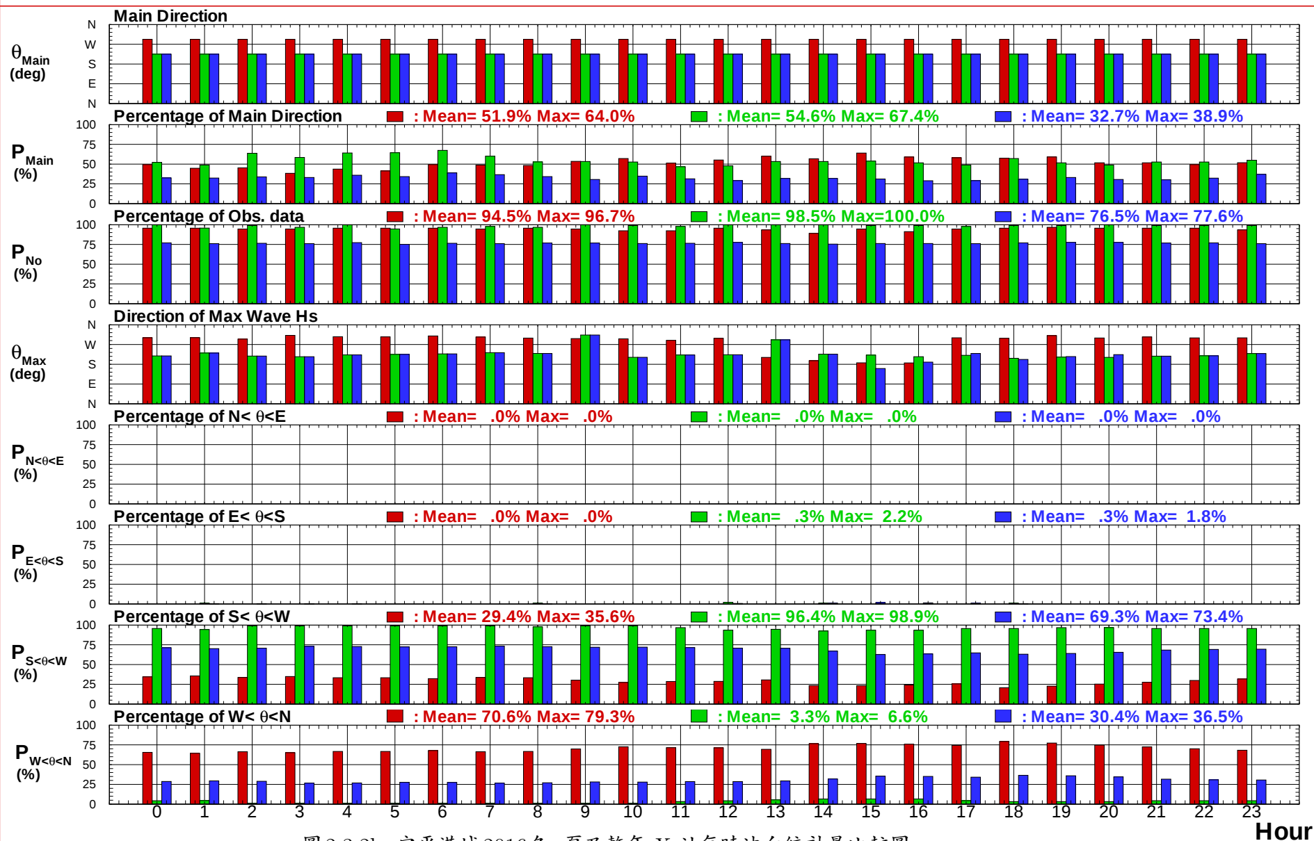
圖 2.3.2b 安平港域2016冬, 夏及整年 X 站每時波向統計量比較圖
