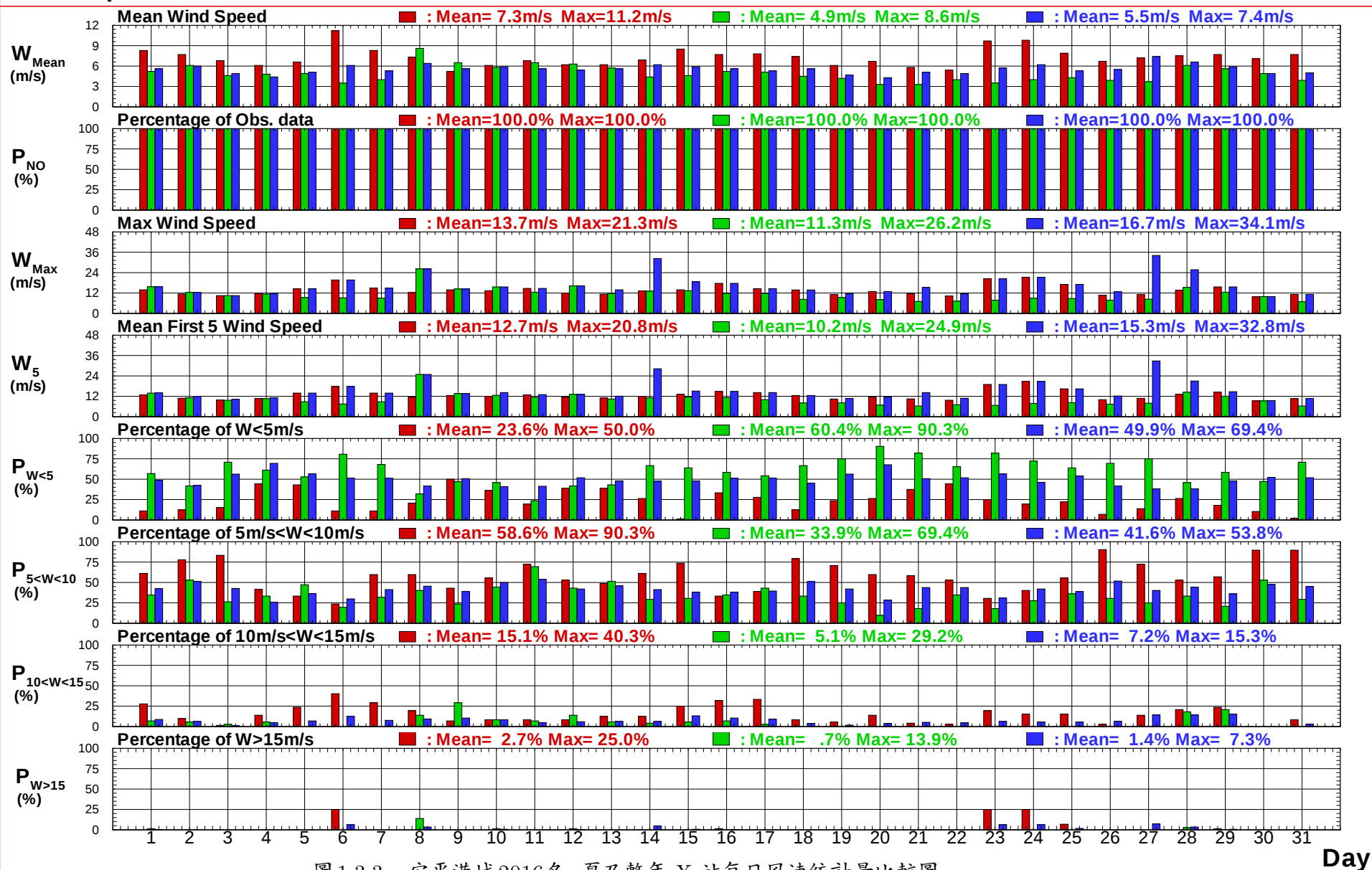
圖 1.3.3a 安平港域2016冬, 夏及整年 X 站每日風速統計量比較圖
