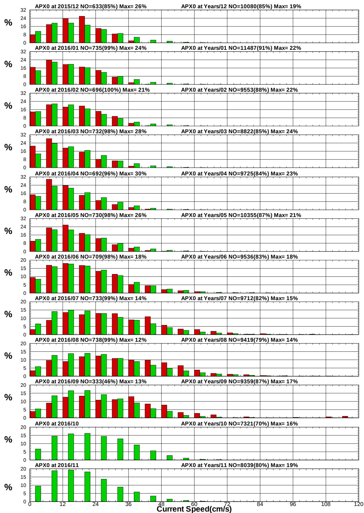
圖 4.3.13a 2016 年及歷年安平港域每月測站 X 流速統計方塊圖
