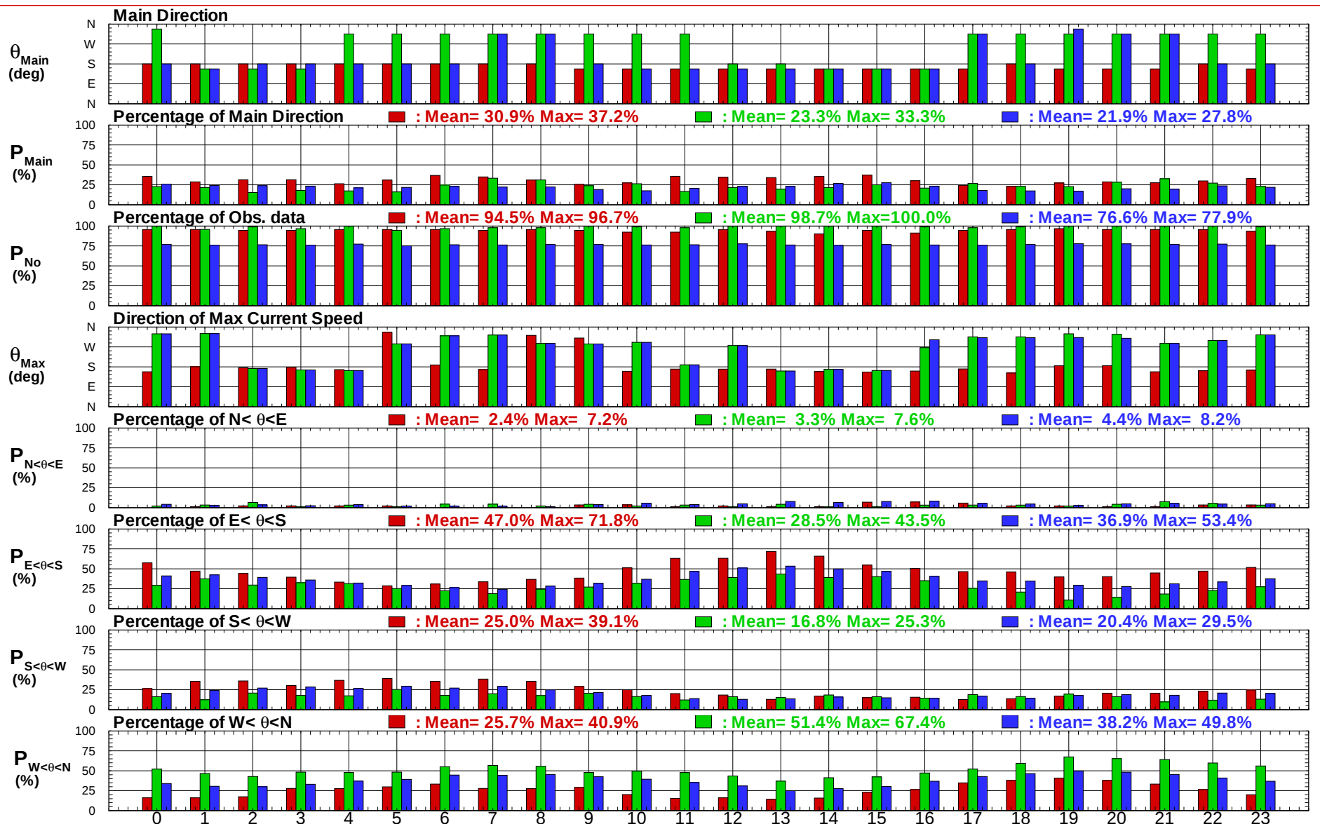
圖 4.3.2b 安平港域2016冬, 夏及整年 X 站逐時流向統計量比較圖
