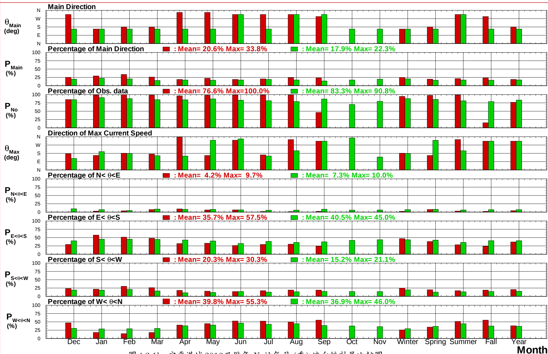
圖 4.3.1b 安平港域 2016 及 歷年 X 站 每月 (季) 流向統計量比較圖
