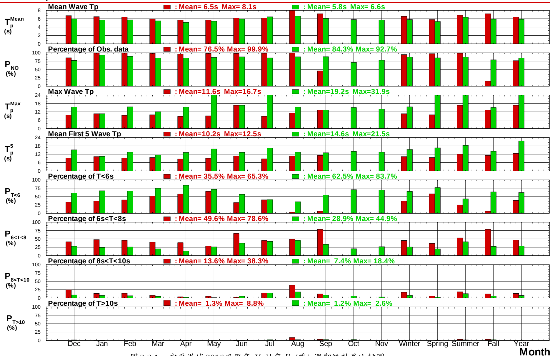
圖 2.3.1c 安平港域 2016 及 歷年 X 站 每月 (季) 週期統計量比較圖
