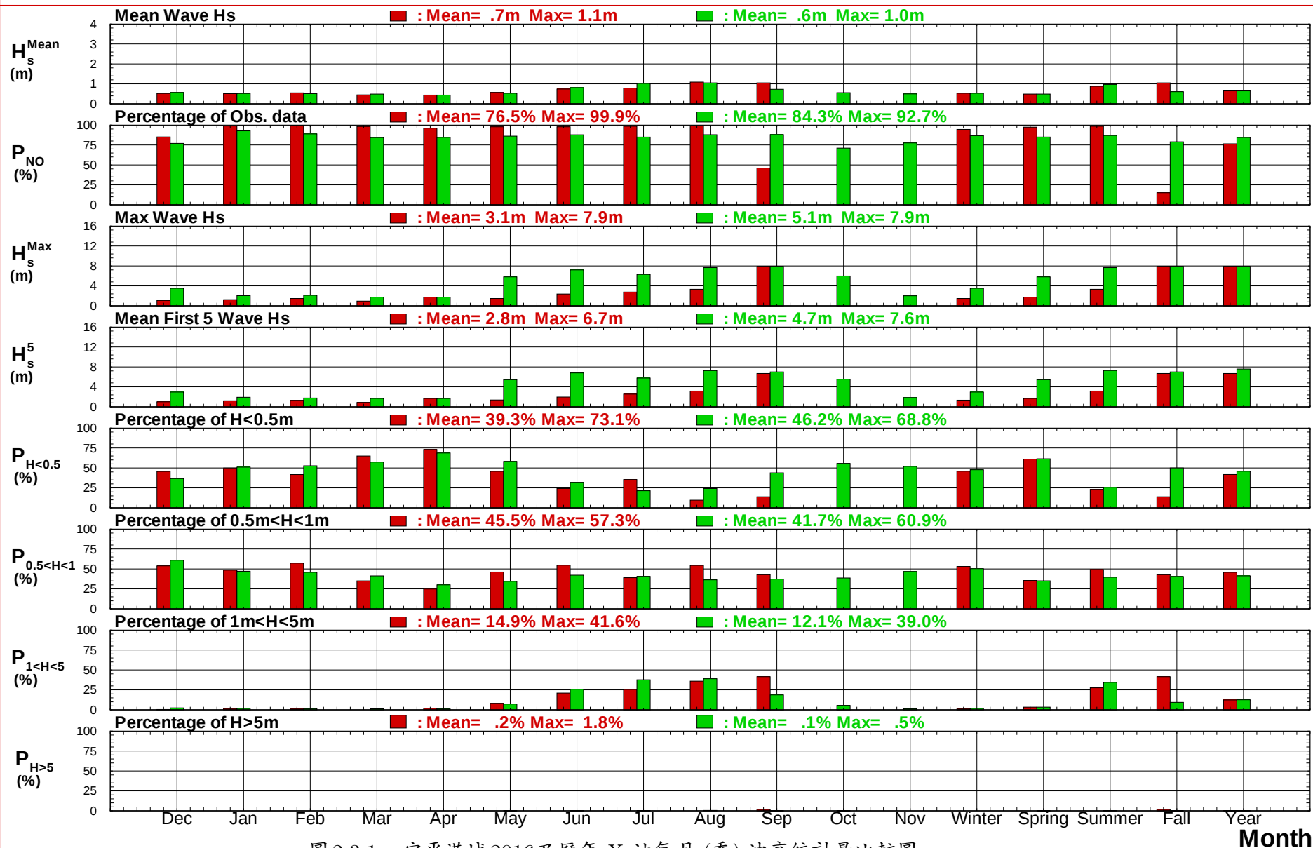
圖 2.3.1a 安平港域2016及歷年 X 站每月 (季) 波高統計量比較圖
