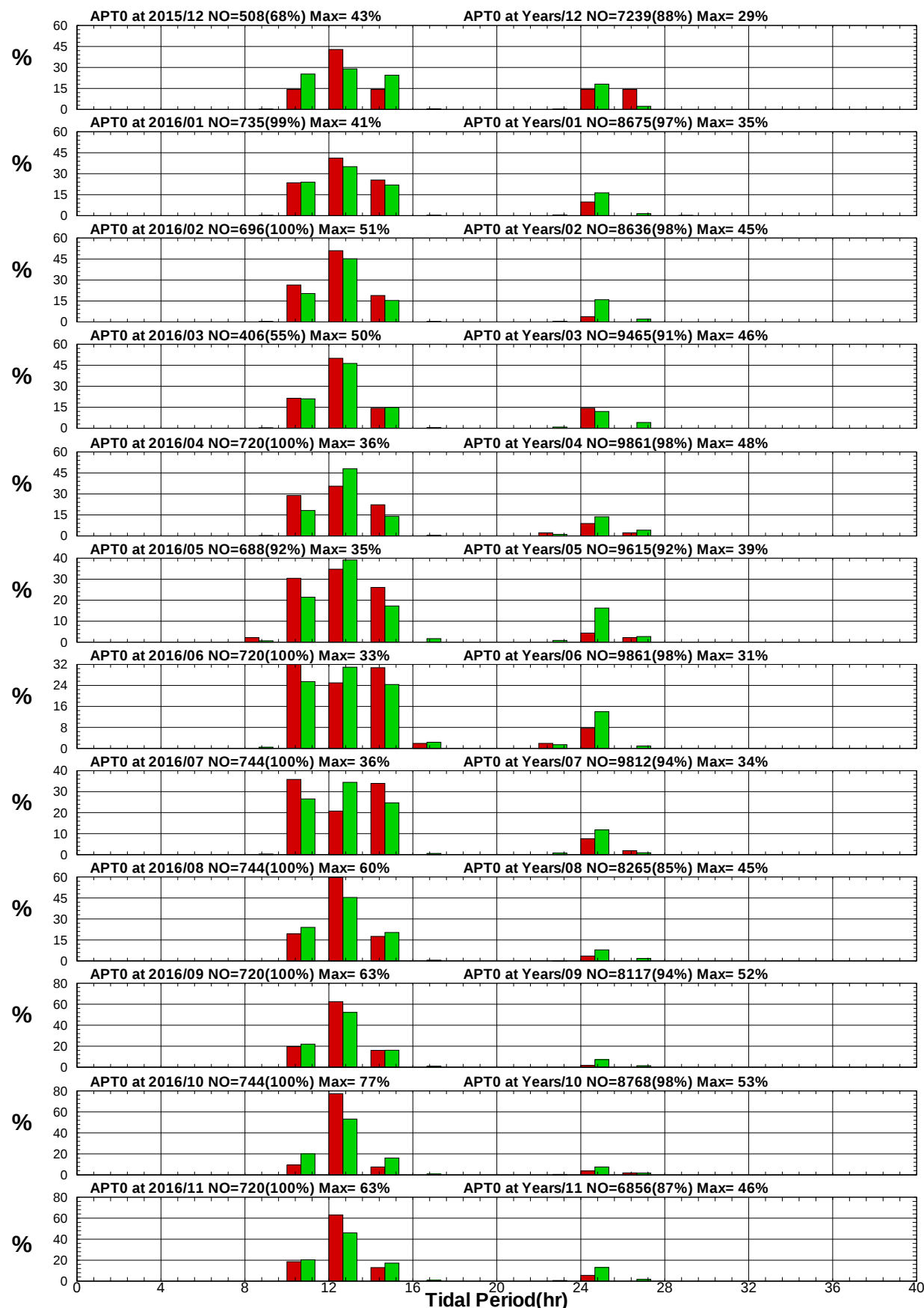
圖 3.3.4e 2016 年及歷年安平港域每月測站 T 週期統計方塊圖
