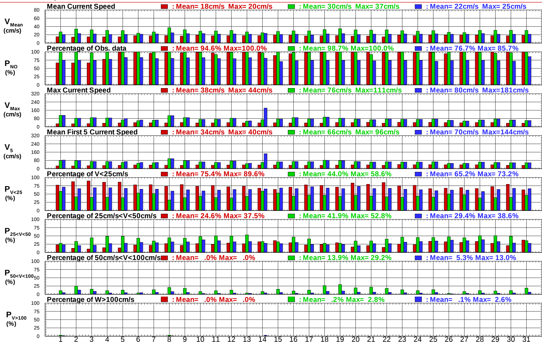
圖 4.3.3a 安平港域2016冬, 夏及整年 X 站每日流速統計量比較圖
