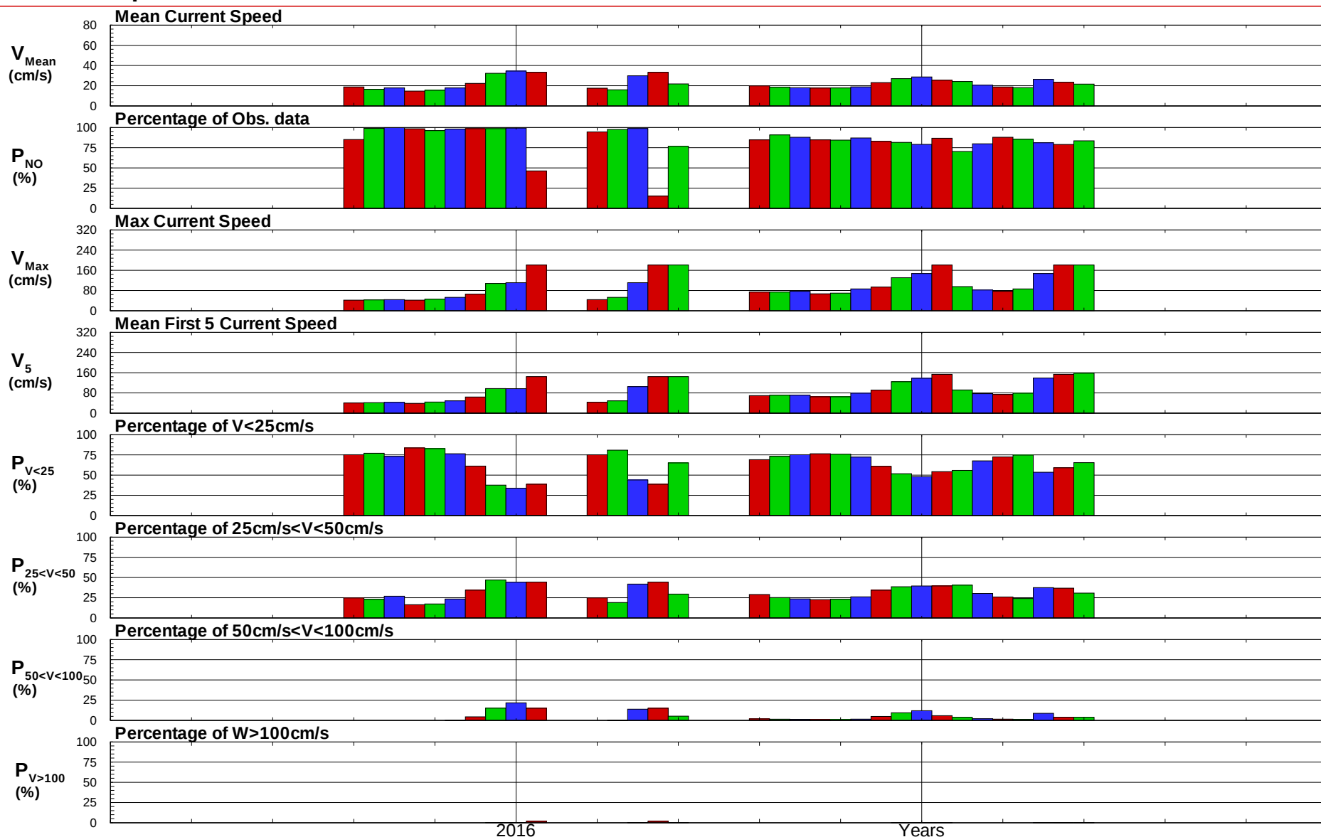
圖 4.3.1c 安平港域 2016 及歷年 X 站每月 (季) 流速統計量比較圖
