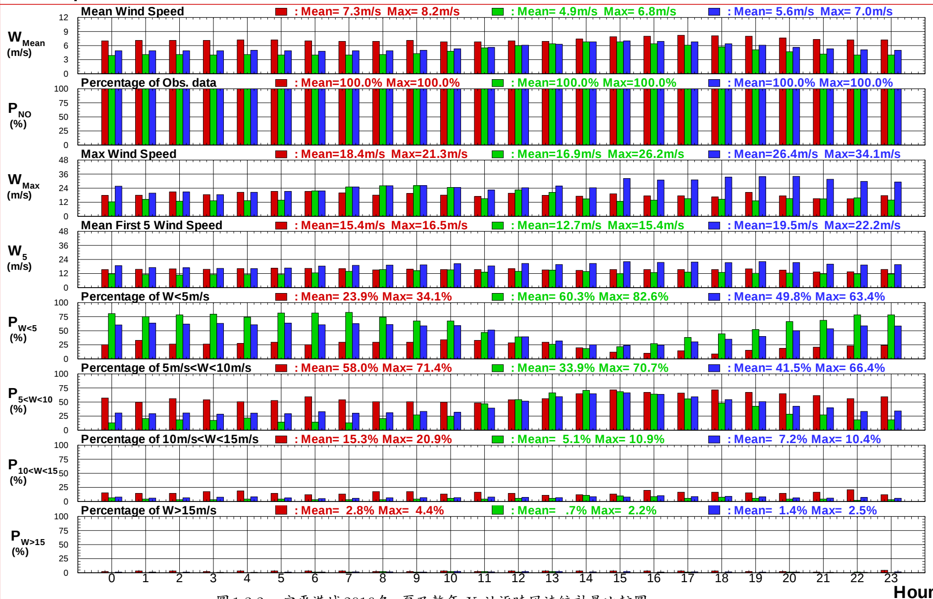
圖 1.3.2a 安平港域2016冬, 夏及整年 X 站逐時風速統計量比較圖
