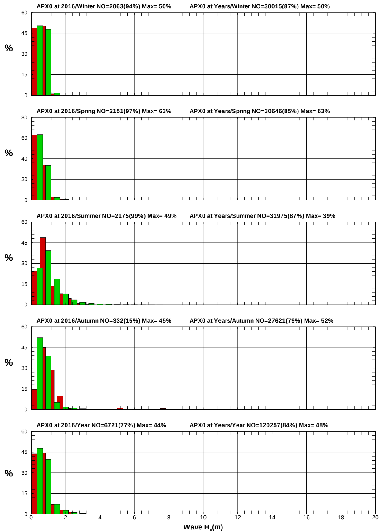
圖 2.3.4b 2016年及歷年安平港域每季測站 X 波高統計方塊圖
