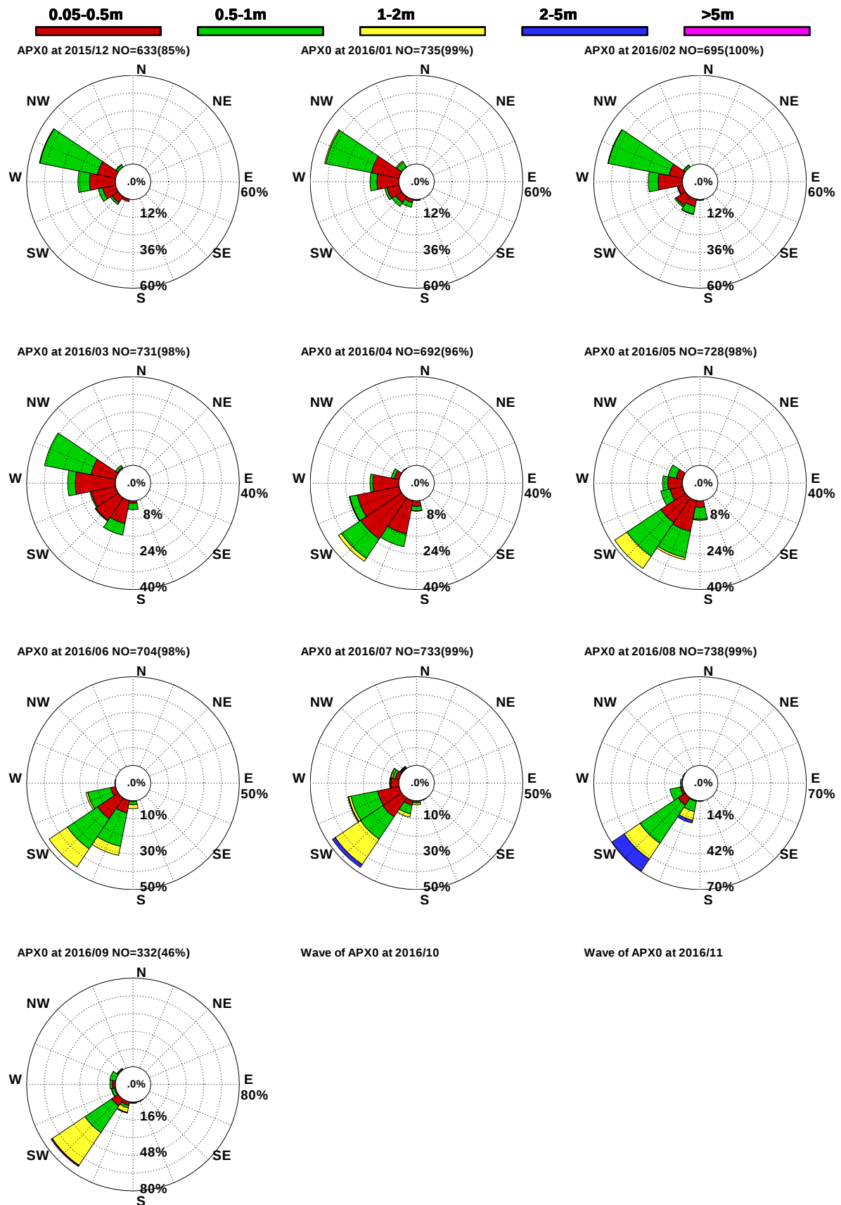
圖 2.3.5a 2016 年安平港域每月測站 X 觀測浪玫瑰圖
