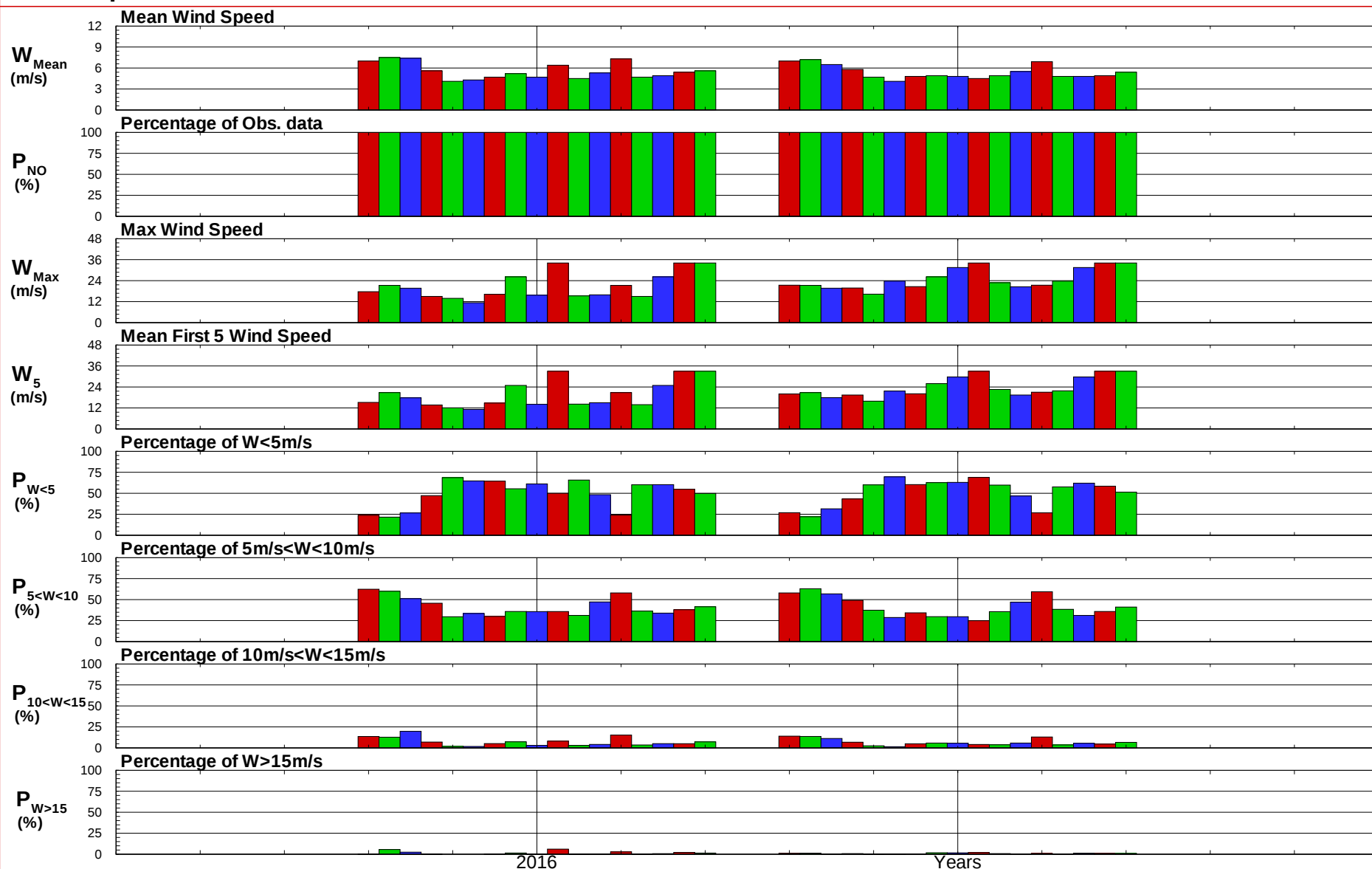
圖 1.3.1c 安平港域 2016 及 歷年 X 站 每 月 (季) 風 速 統 計 量 比 較 圖
