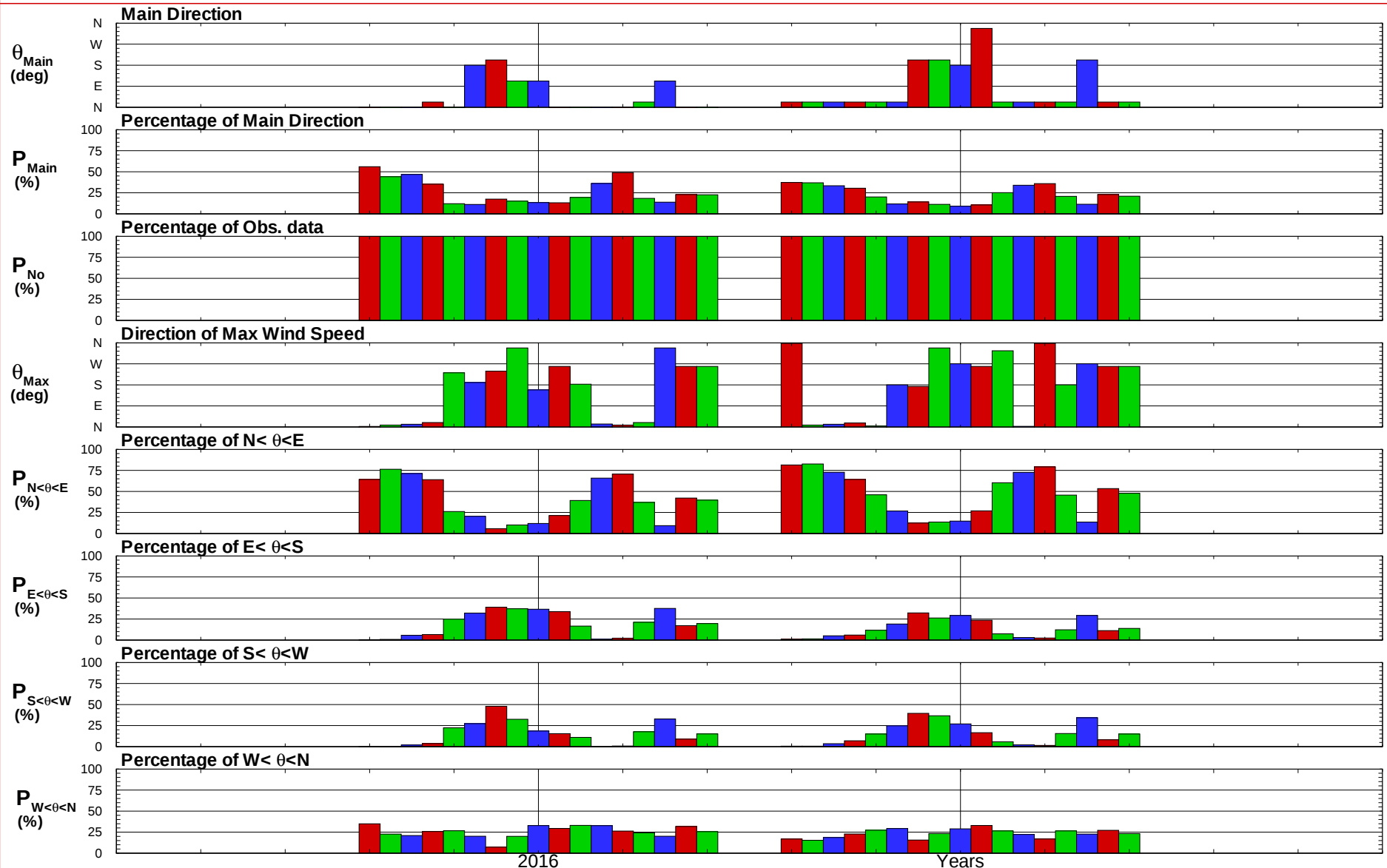
圖 1.3.1d 安平港域 2016 及歷年 X 站每月 (季) 風向統計量比較圖
