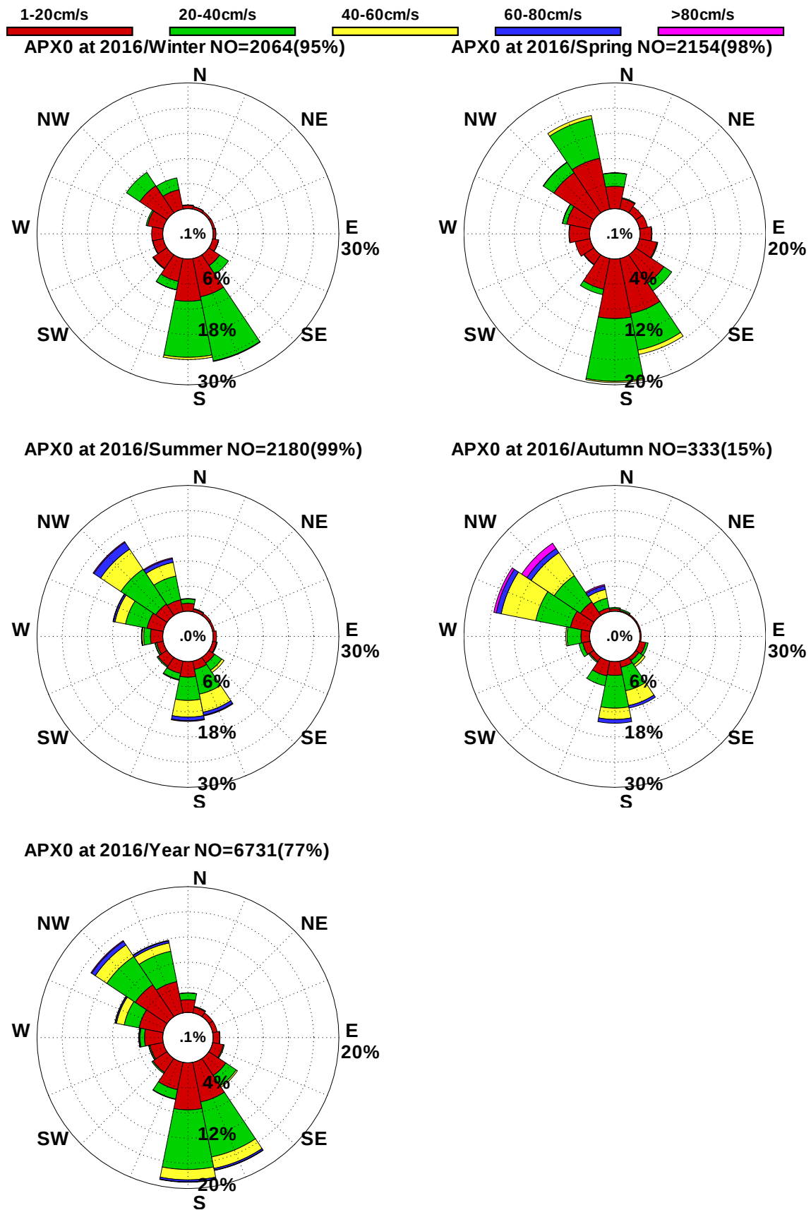
圖 4.3.5b 2016 年安平港域每季測站 X 觀測流玫瑰圖
