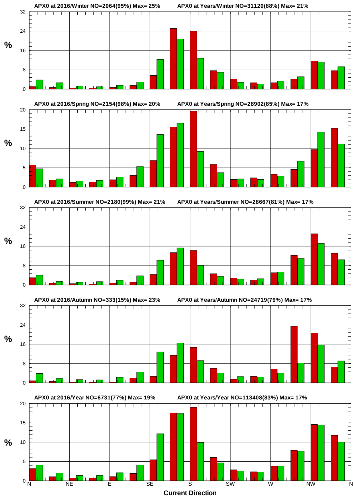
圖 4.3.16d 2016 年及歷年安平港域每季測站 X 流向統計方塊圖
