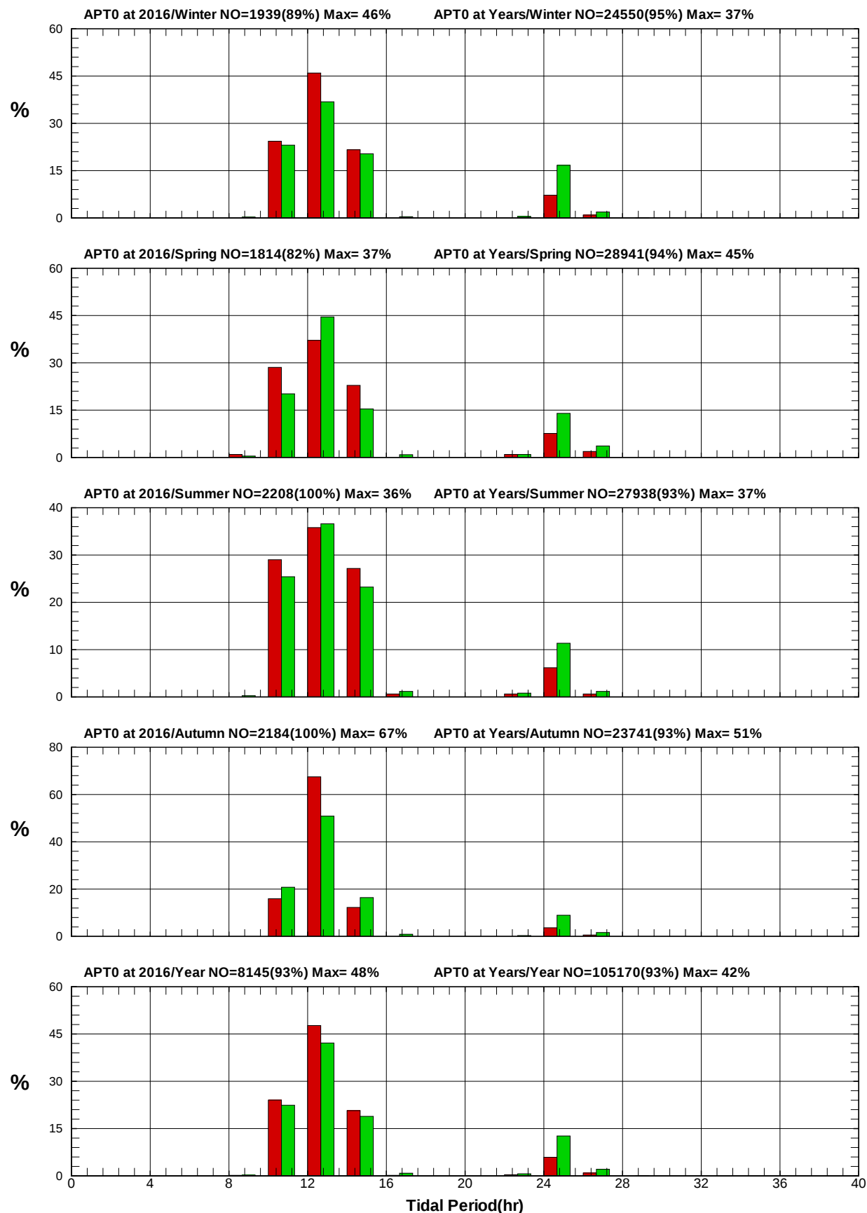
圖 3.3.4f 2016 年及歷年安平港域每季測站 T 週期統計方塊圖
