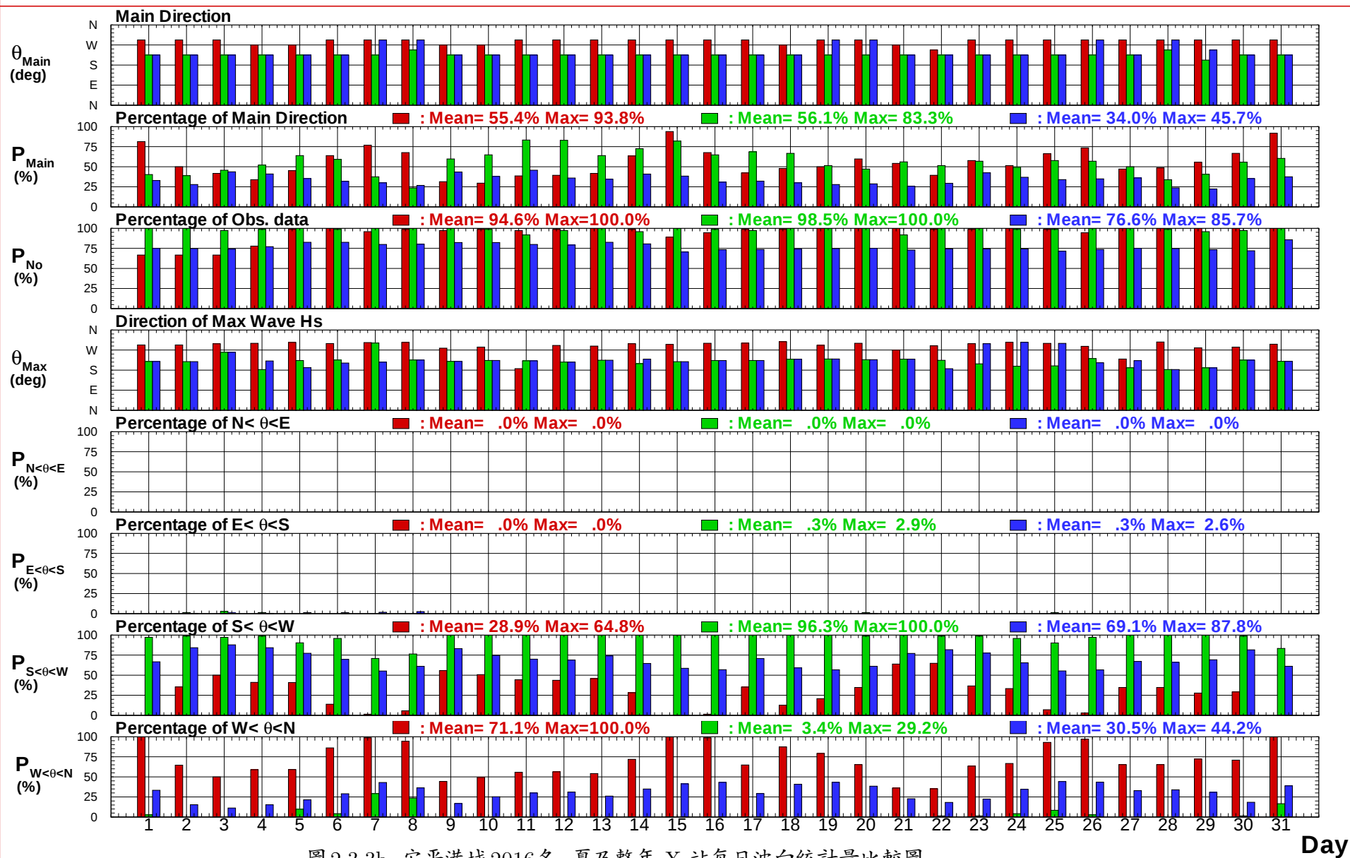
圖 2.3.3b 安平港域2016冬, 夏及整年 X 站每日波向統計量比較圖
