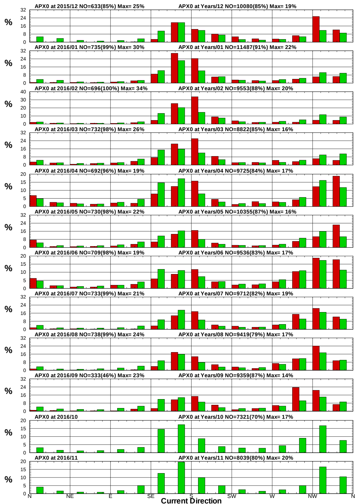
圖 4.3.15c 2016 年及歷年安平港域每月測站 X 流向統計方塊圖
