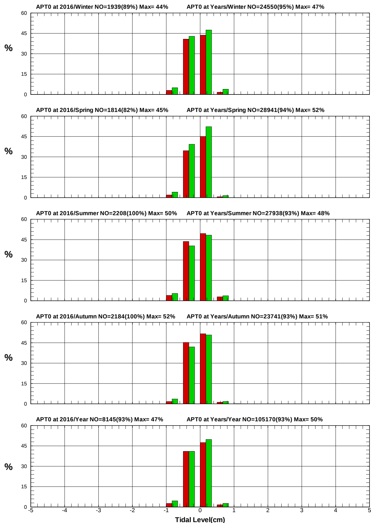
圖 3.3.4b 2016年及歷年安平港域每季測站 T 潮位統計方塊圖
