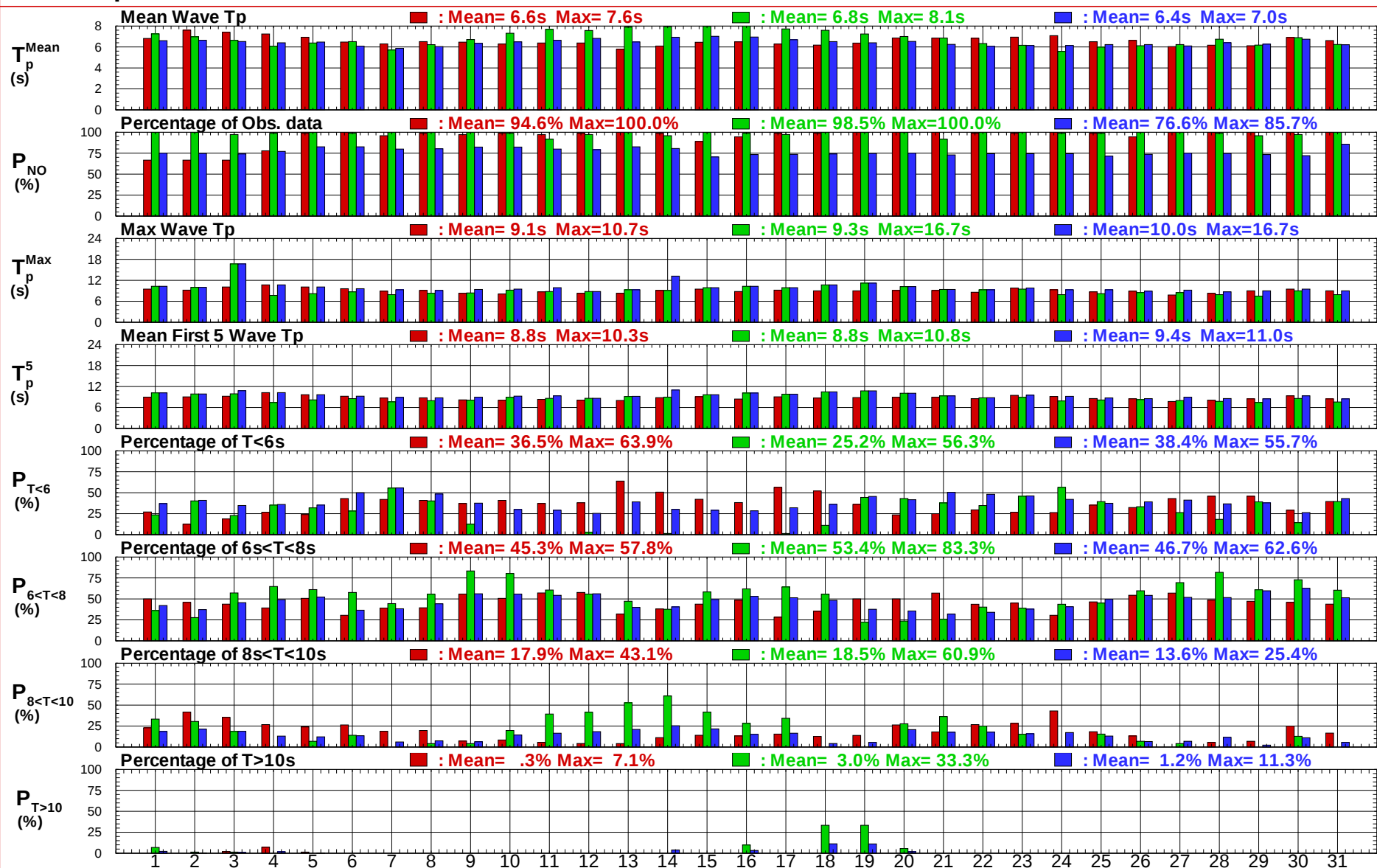
圖 2.3.3c 安平港域2016冬,夏及整年 X 站每日週期統計量比較圖
