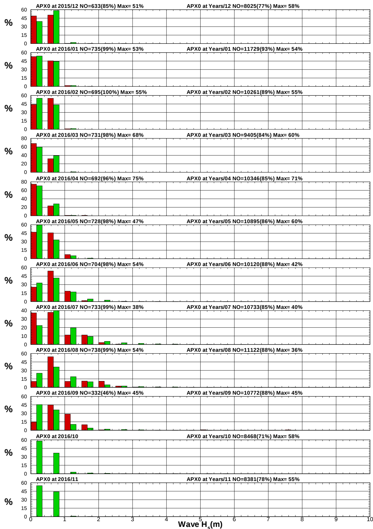
圖 2.3.4a 2016 年及歷年安平港域每月測站 X 波高統計方塊圖
