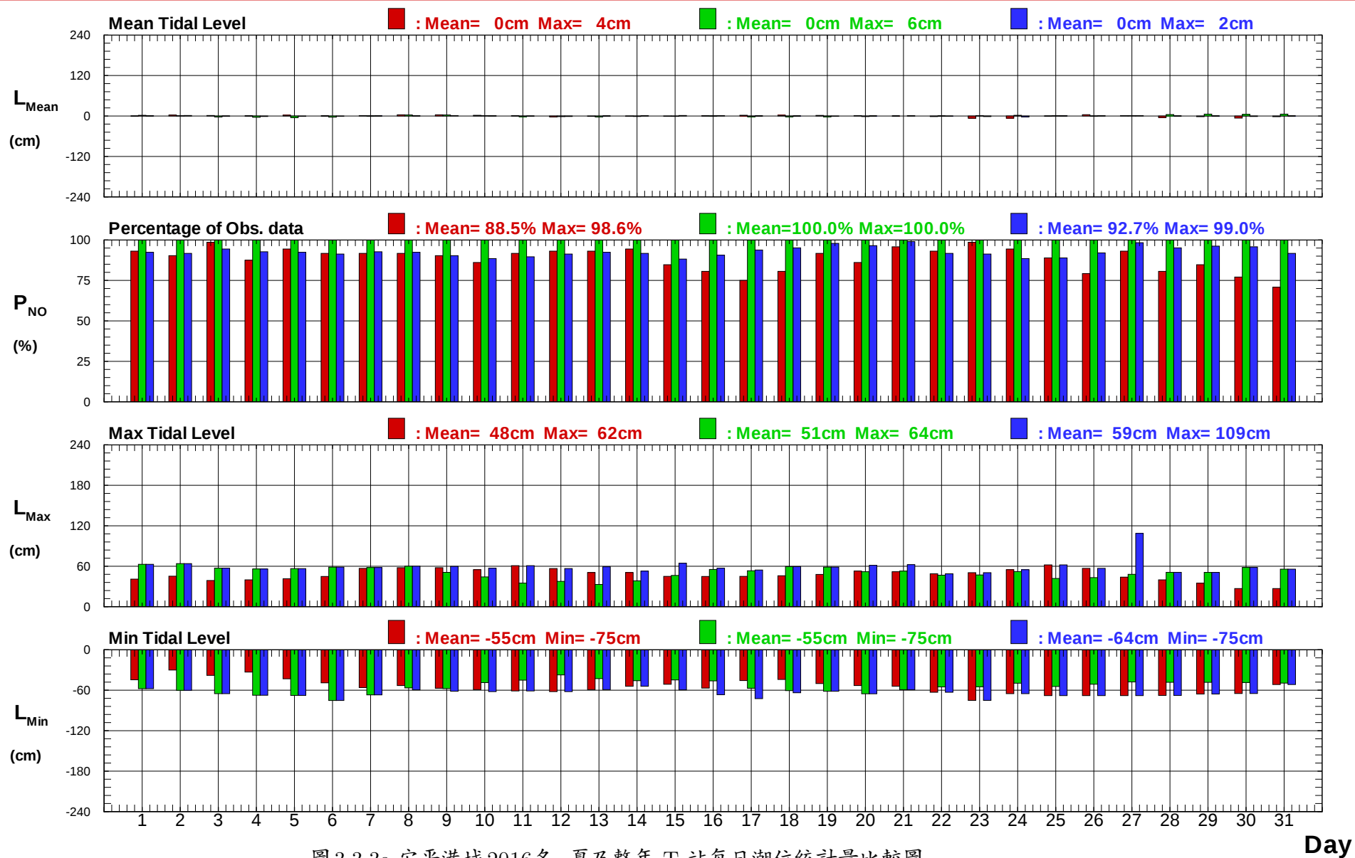
圖 3.3.3a 安平港域 2016 冬、夏及整年 T 站每日潮位統計量比較圖
