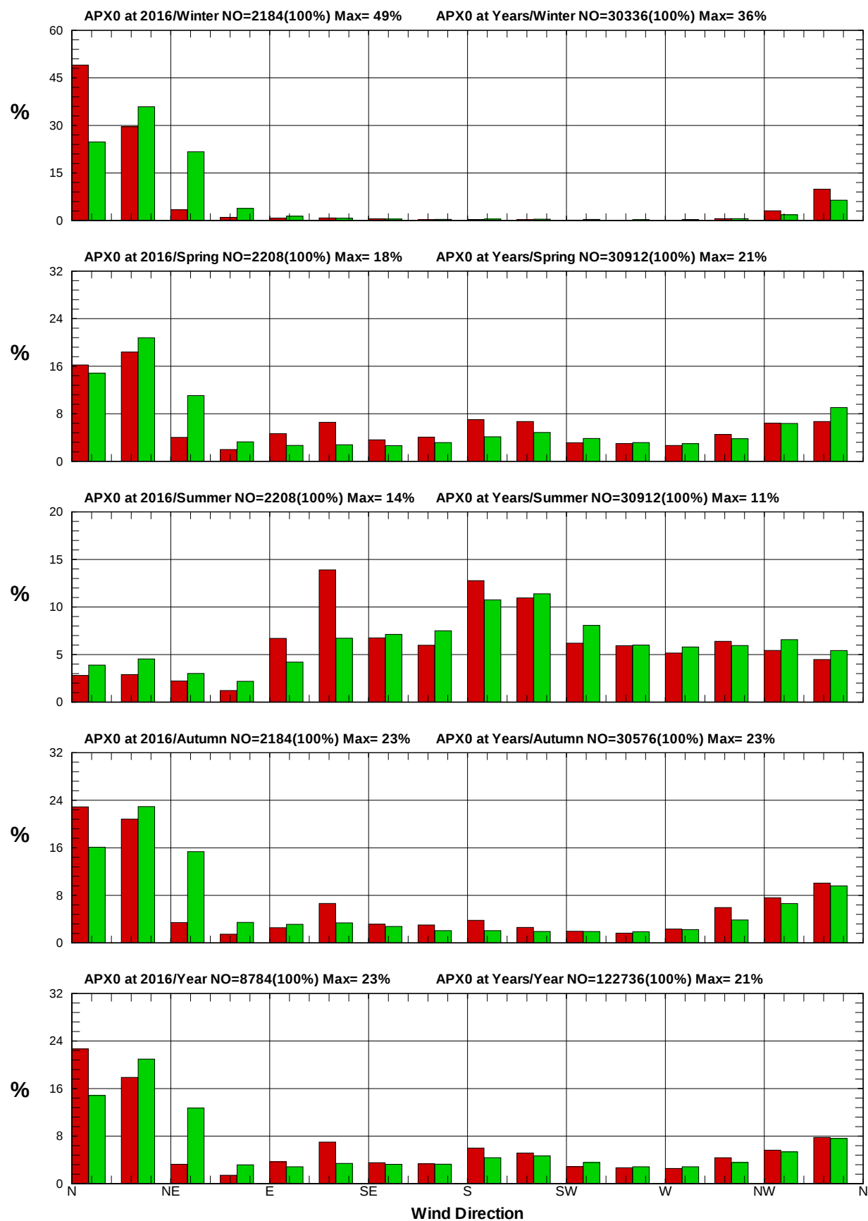
圖 1.3.4d 2016年及歷年安平港域每季測站 X 風向統計方塊圖
