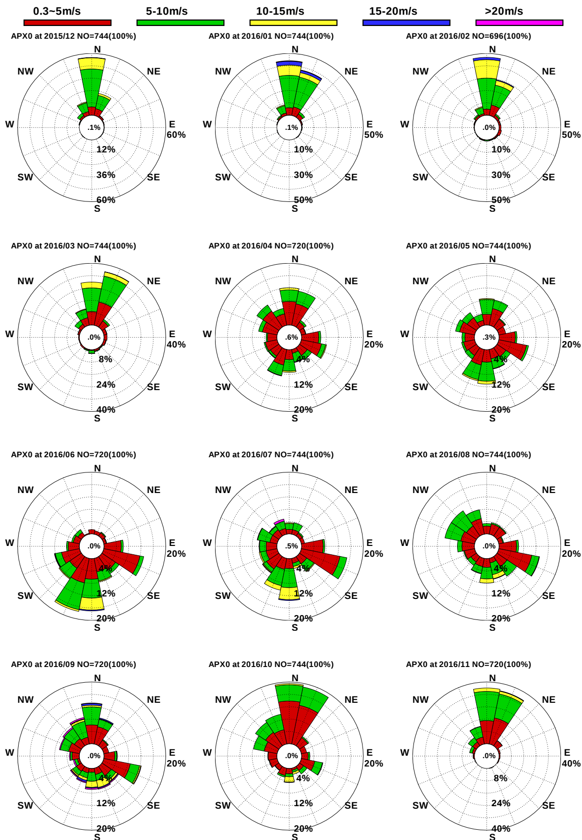
圖 1.3.5a 2016 年安平港域每月測站 X 觀測風玫瑰圖
