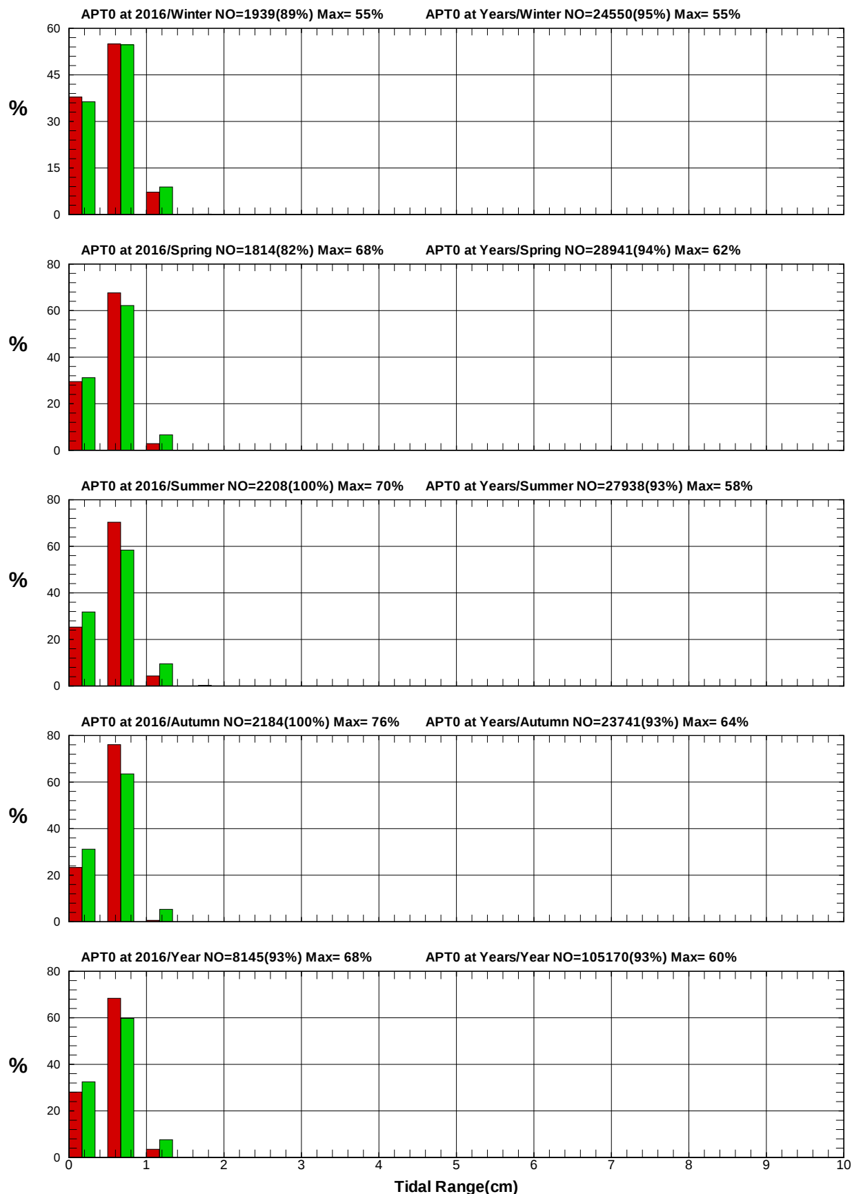
圖 3.3.4d 2016年及歷年安平港域每季測站 T 潮差統計方塊圖
