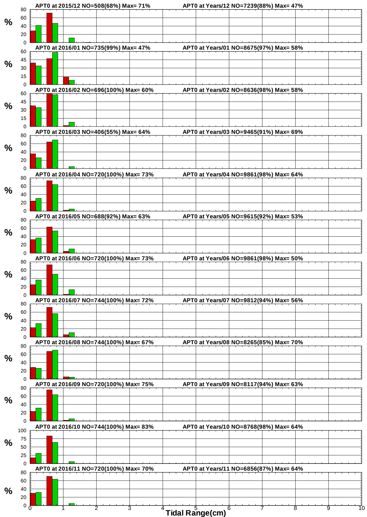
圖 3.3.4c 2016 年及歷年安平港域每月測站 T 潮差統計方塊圖
