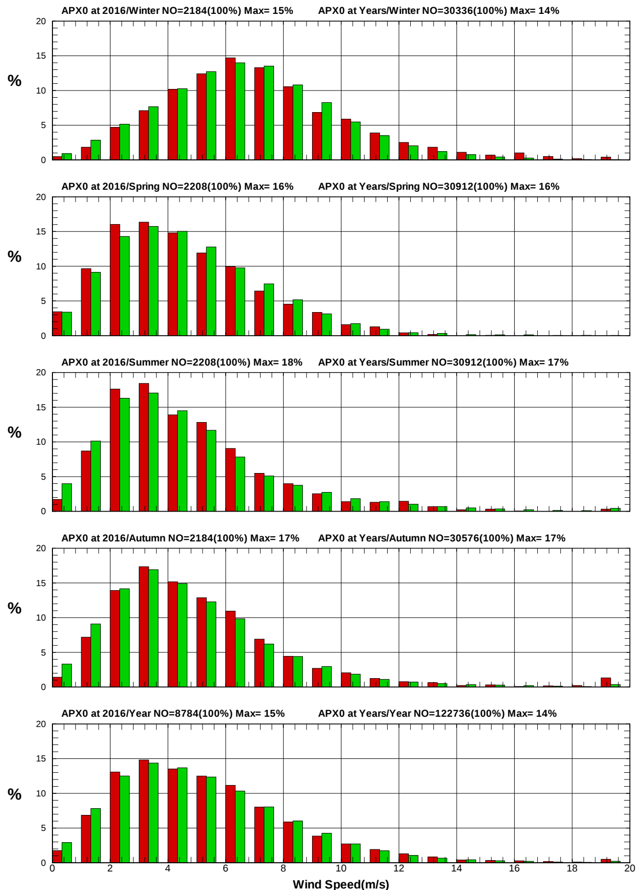
圖 1.3.4b 2016年及歷年安平港域每季測站 X 風速統計方塊圖
