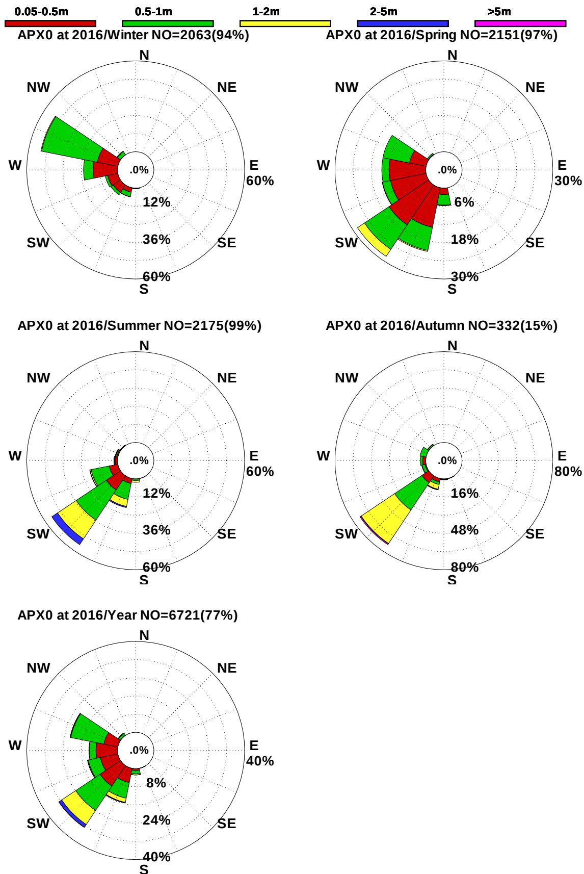
圖 2.3.5b 2016 年安平港域每季測站 X 觀測浪玫瑰圖
