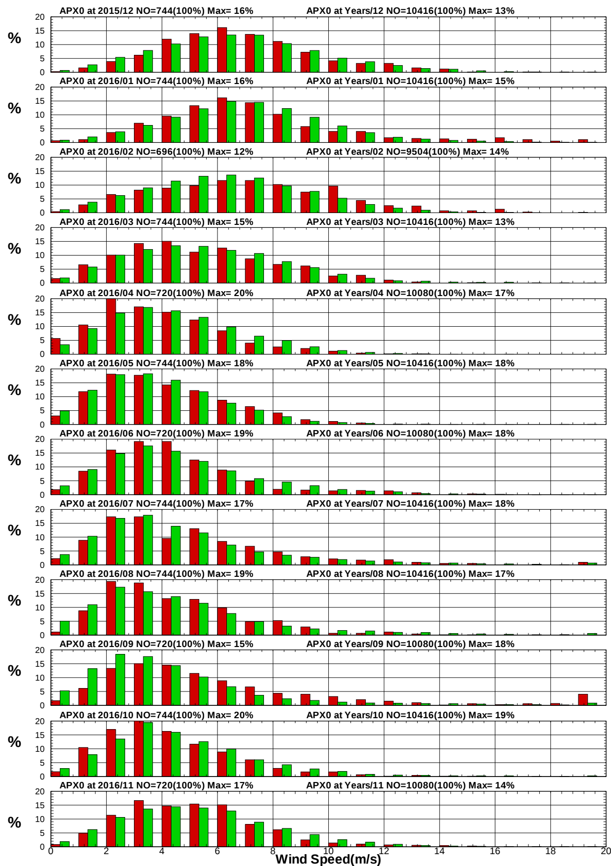
圖 1.3.4a 2016 年及歷年安平港域每月測站 X 風速統計方塊圖
