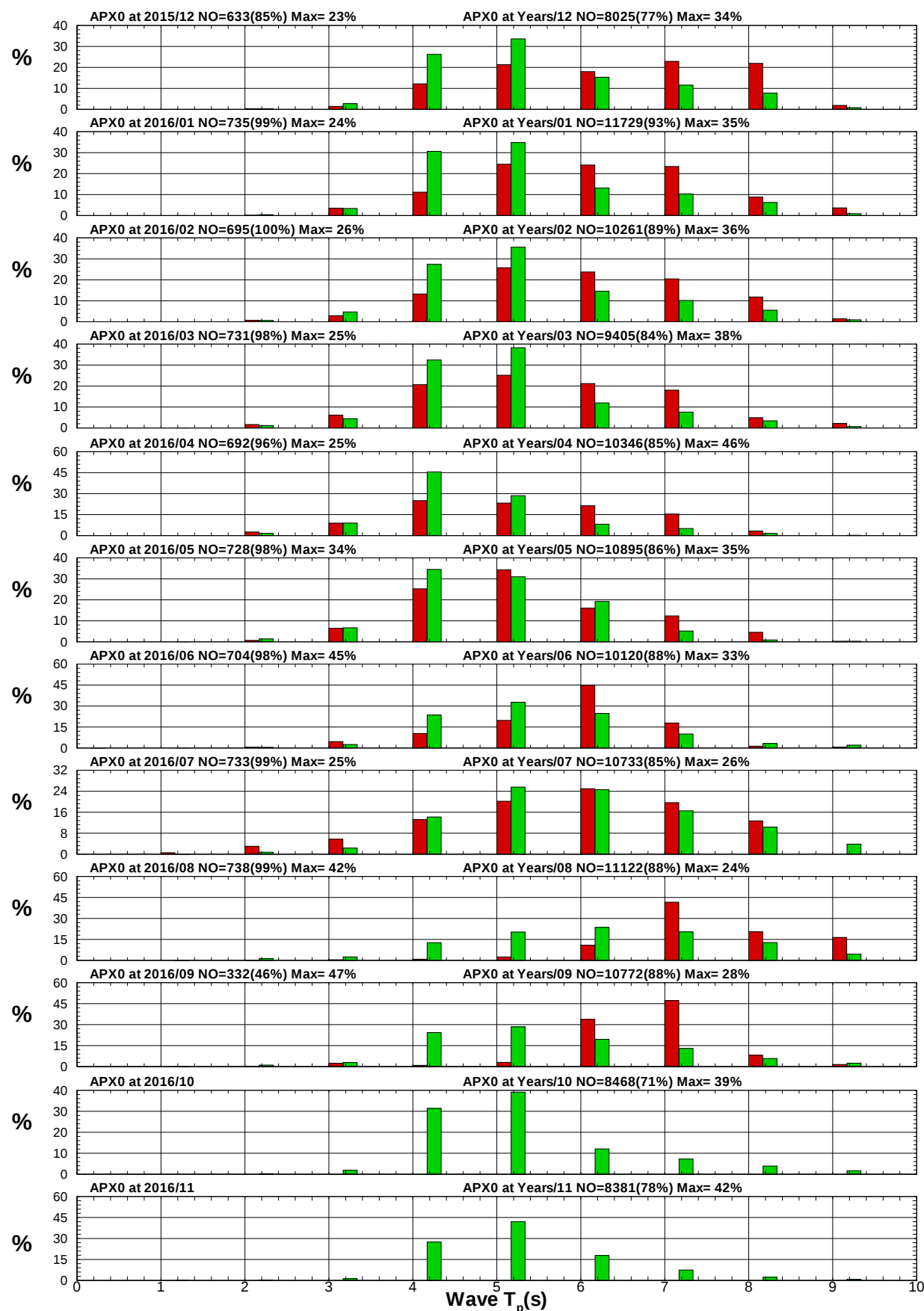
圖 2.3.4e 2016 年及歷年安平港域每月測站 X 週期統計方塊圖
