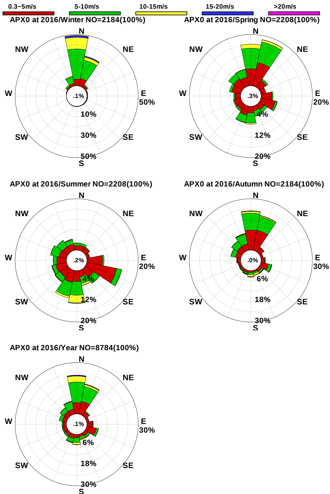
圖 1.3.5b 2016 年安平港域每季測站 X 觀測風玫瑰圖
