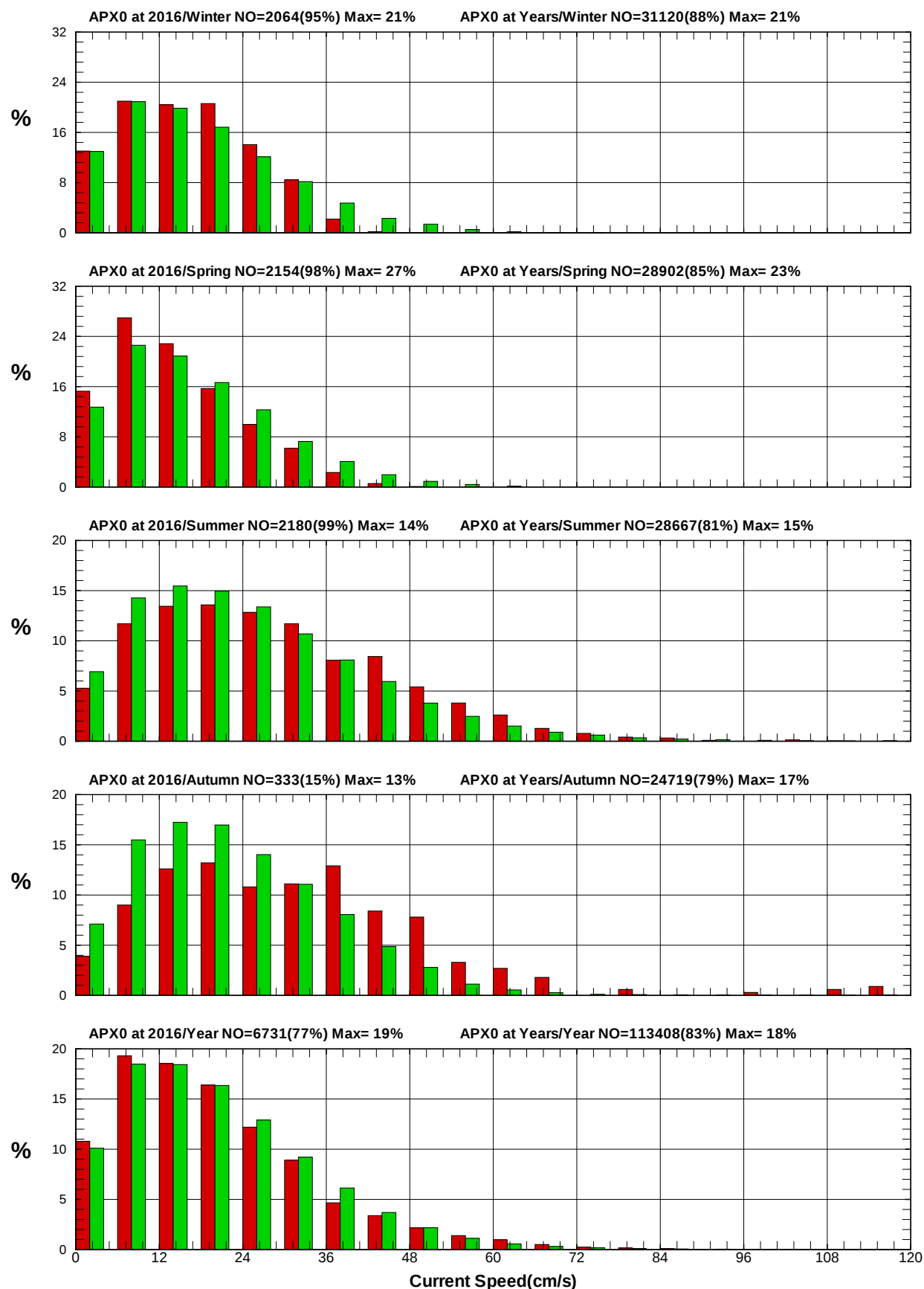
圖 4.3.14b 2016 年及歷年安平港域每季測站 X 流速統計方塊圖
