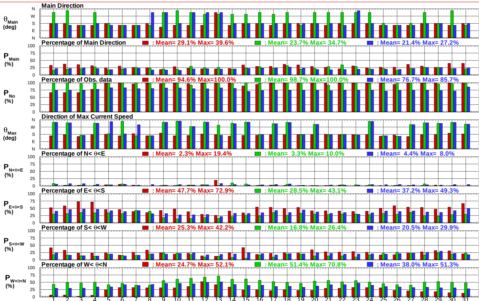
圖 4.3.3b 安平港域2016冬, 夏及整年 X 站每日流向統計量比較圖
