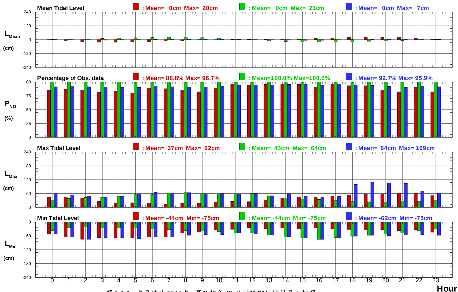
圖 3.3.2a 安平港域 2016 冬、夏及整年 T 站逐時潮位統計量比較圖
