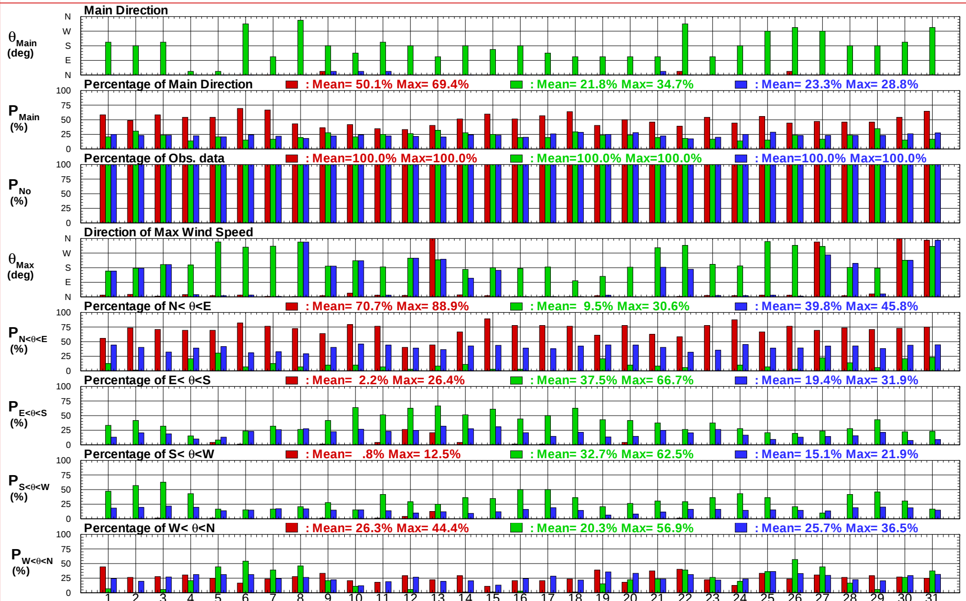
圖 1.3.3b 安平港域2016冬, 夏及整年 X 站每日風向統計量比較圖
