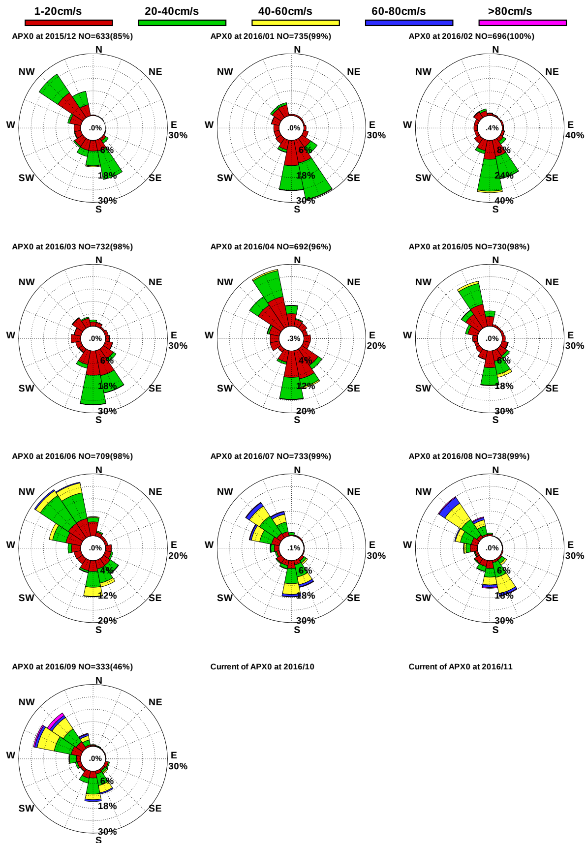
圖 4.3.5a 2016 年安平港域每月測站 X 觀測流玫瑰圖
