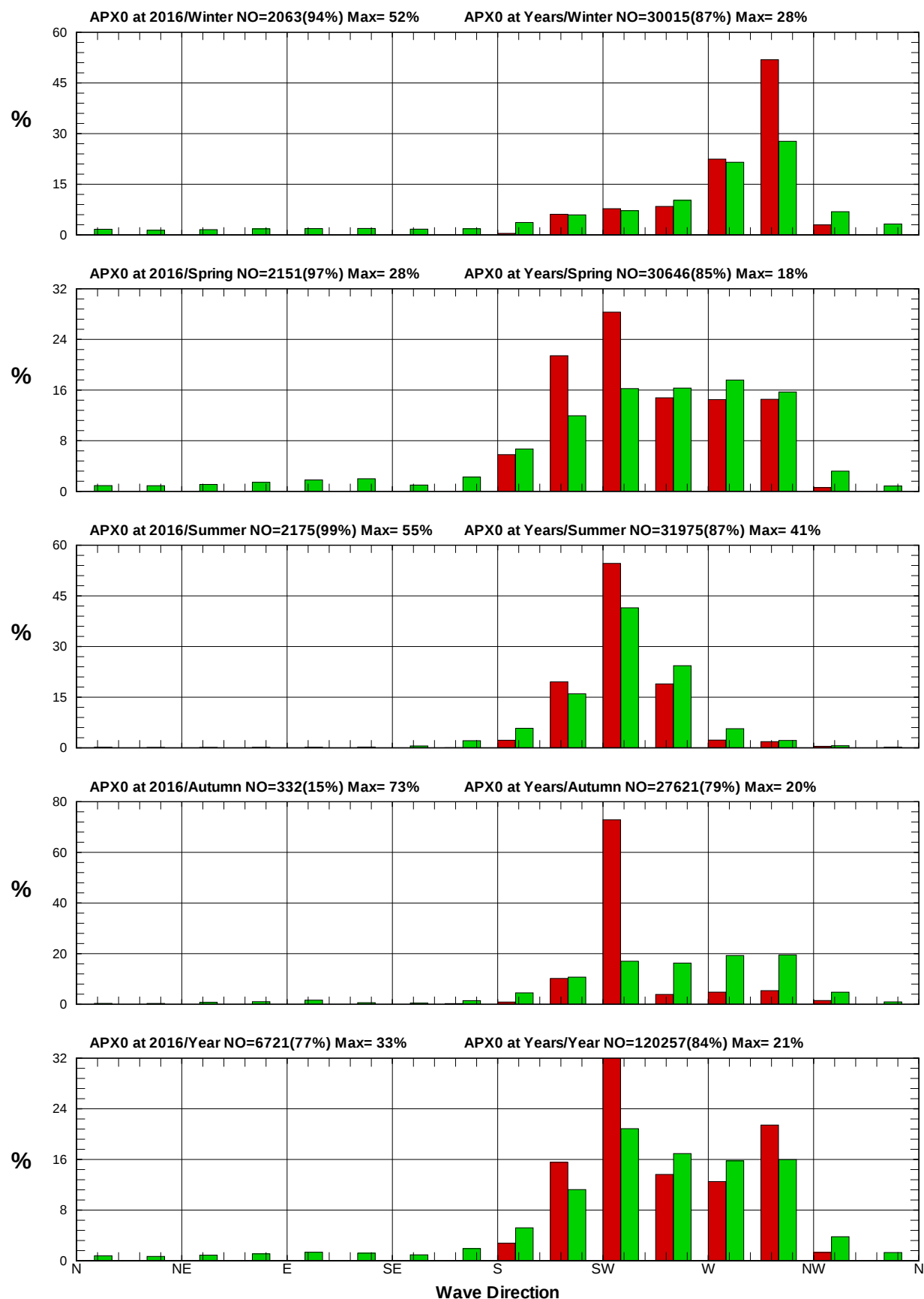
圖 2.3.4d 2016年及歷年安平港域每季測站 X 波向統計方塊圖
