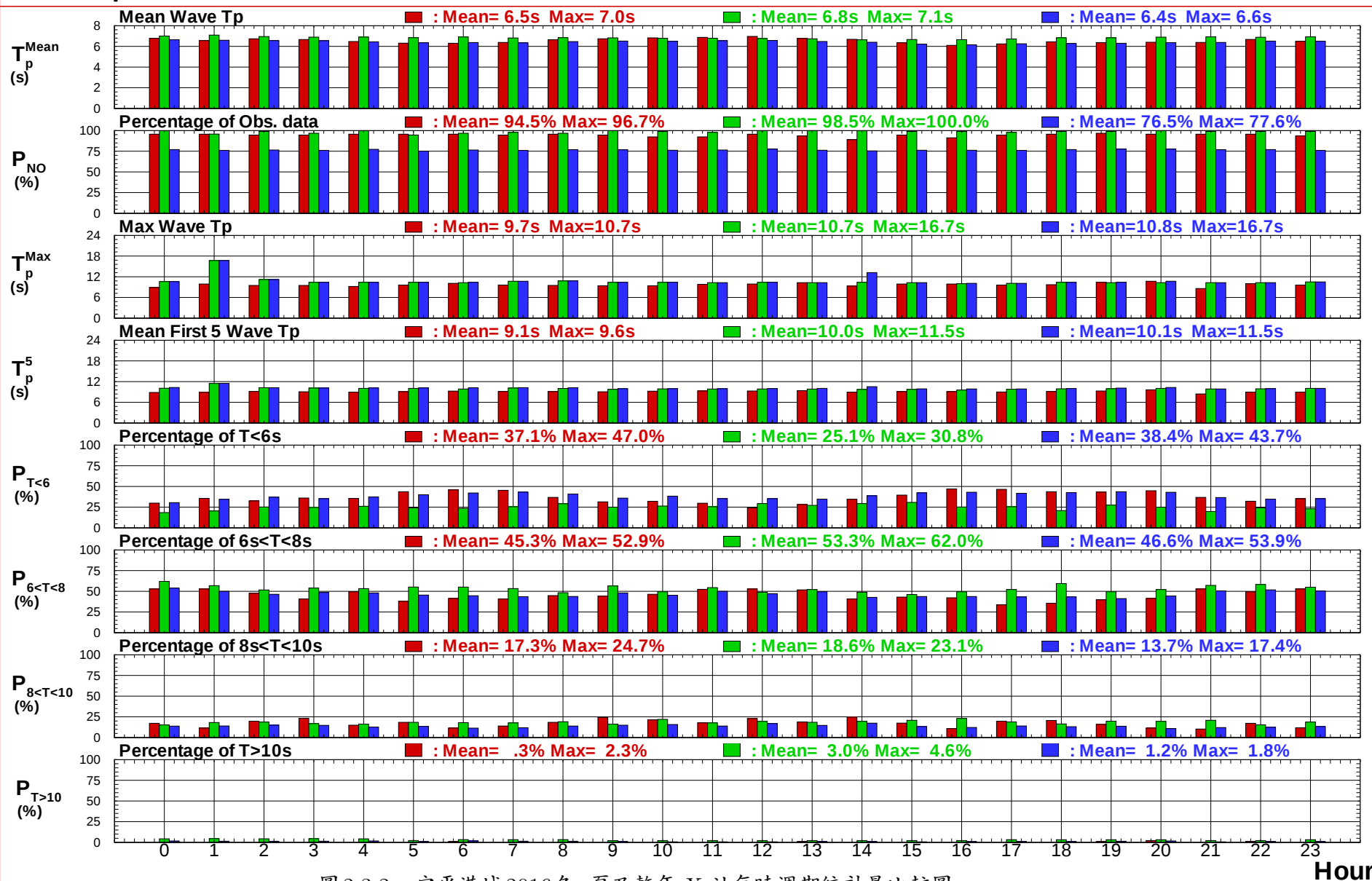
圖 2.3.2c 安平港域2016冬,夏及整年 X 站每時週期統計量比較圖
