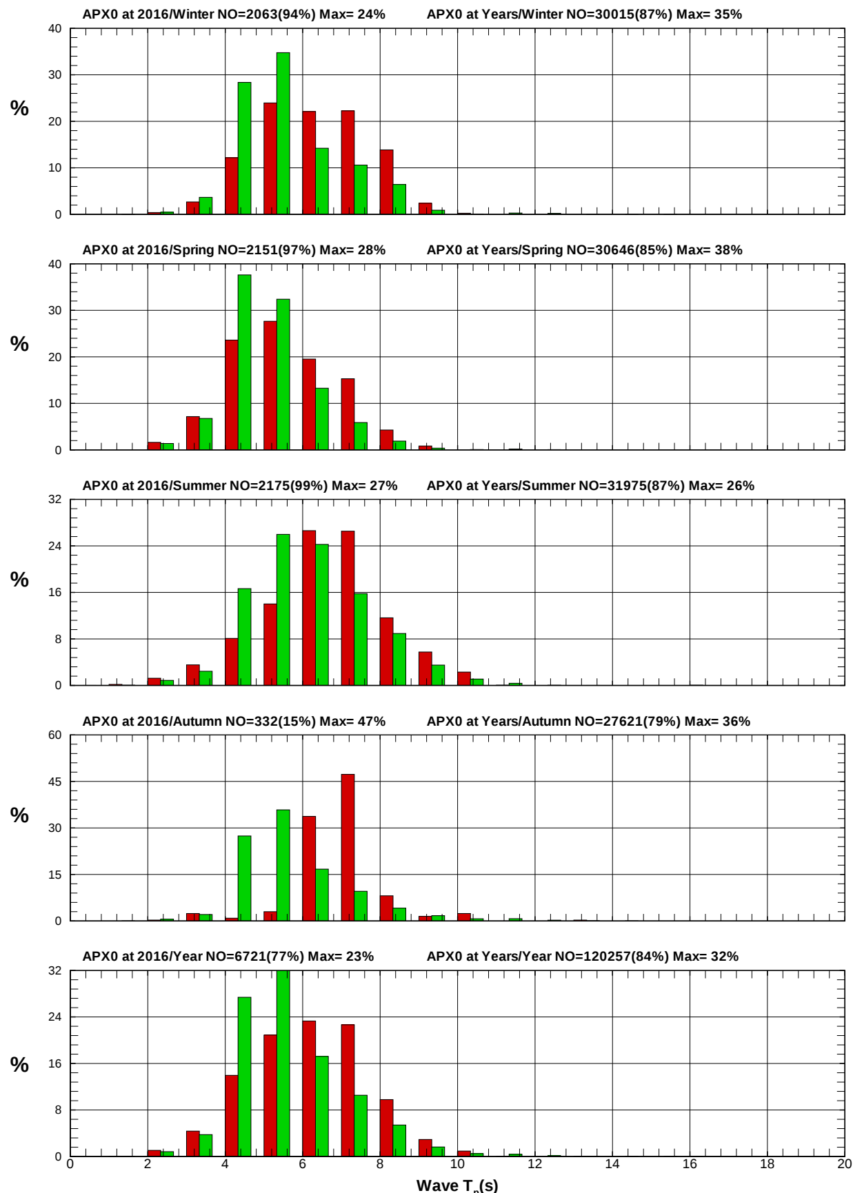
圖 2.3.4f 2016 年及歷年安平港域每季測站 X 週期統計方塊圖
