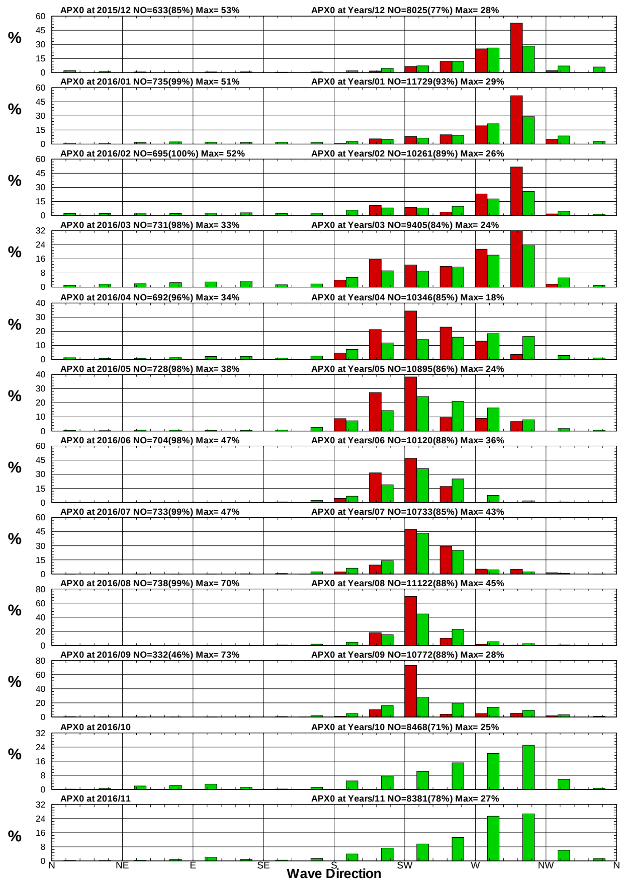
圖 2.3.4c 2016 年及歷年安平港域每月測站 X 波向統計方塊圖
