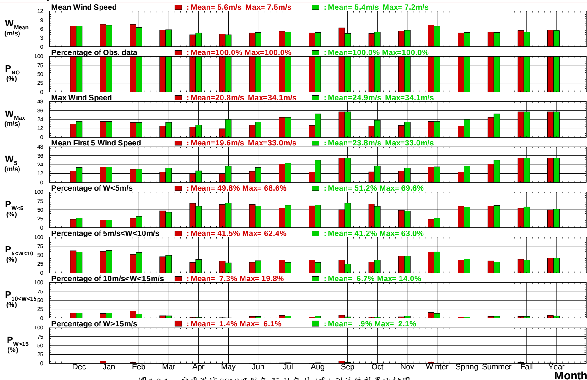
圖 1.3.1a 安平港域 2016 及 歷年 X 站 每月 (季) 風速統計量比較圖
