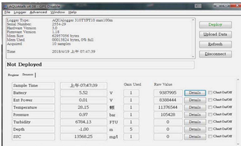
圖3.2.5 AQUAtalk 與 AQUAlogger 310TY之操作畫面二
