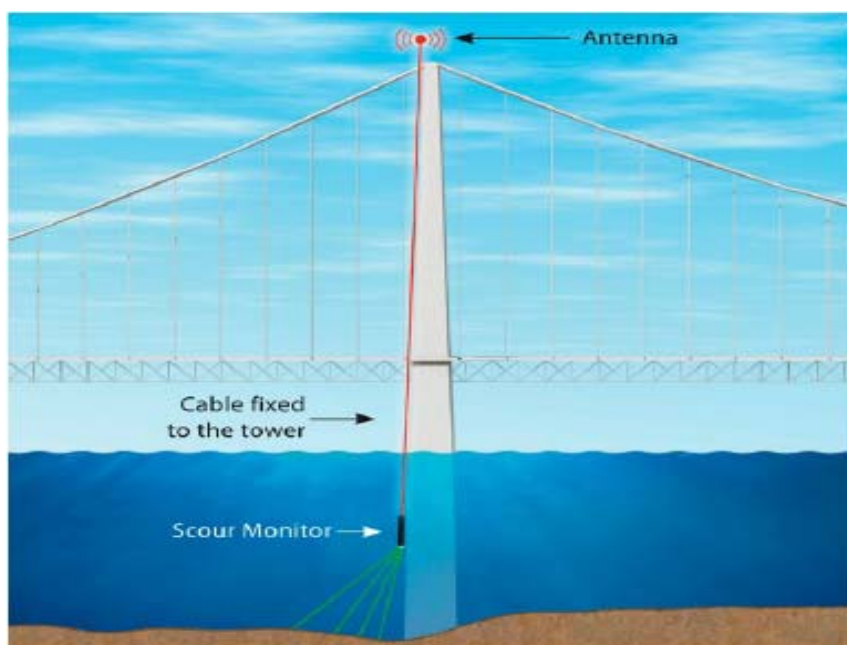
圖5.2.1 淘刷監測儀安裝於橋梁示意圖
