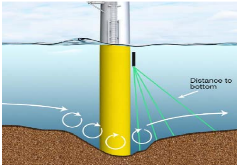
圖5.2.2 淘刷監測儀安裝於單樁(monopiles)示意圖
