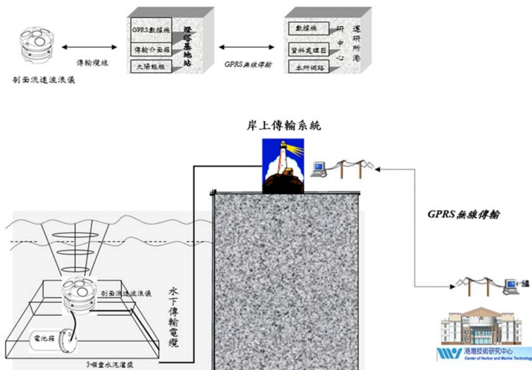
圖4.2.5 底碇式水下波流及海流觀測系統
