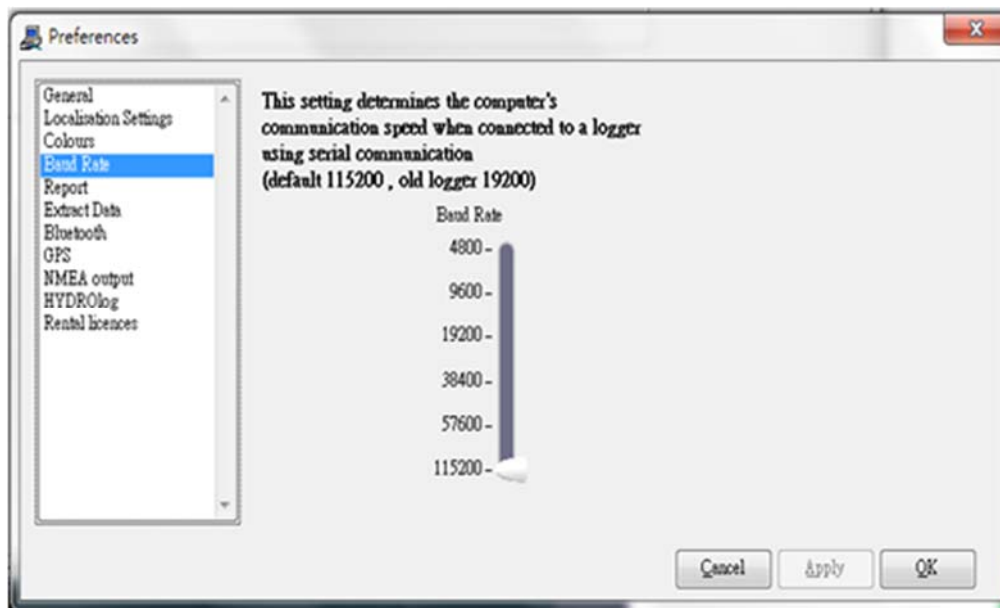
圖3.2.6 AQUAtalk 與 AQUAlogger 310TY之操作畫面三
