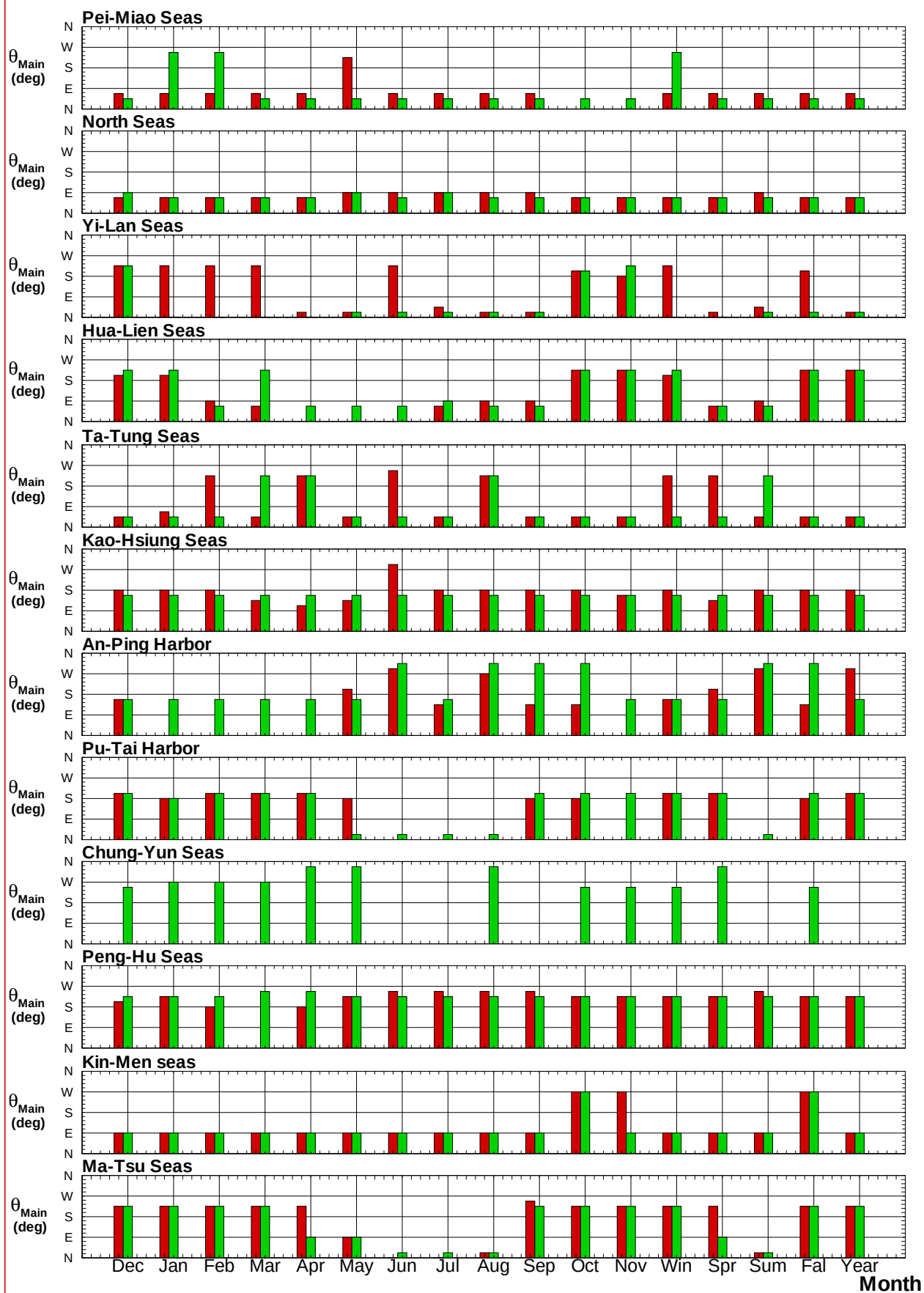
圖7.3e 2017及歷年12港域主要測站每月(季)主要流向比較圖
