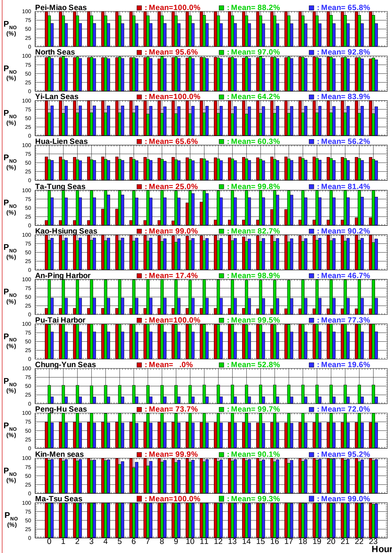
圖7.4b 2017年12港域冬, 夏及整年主要測站逐時蒐集率比較圖
