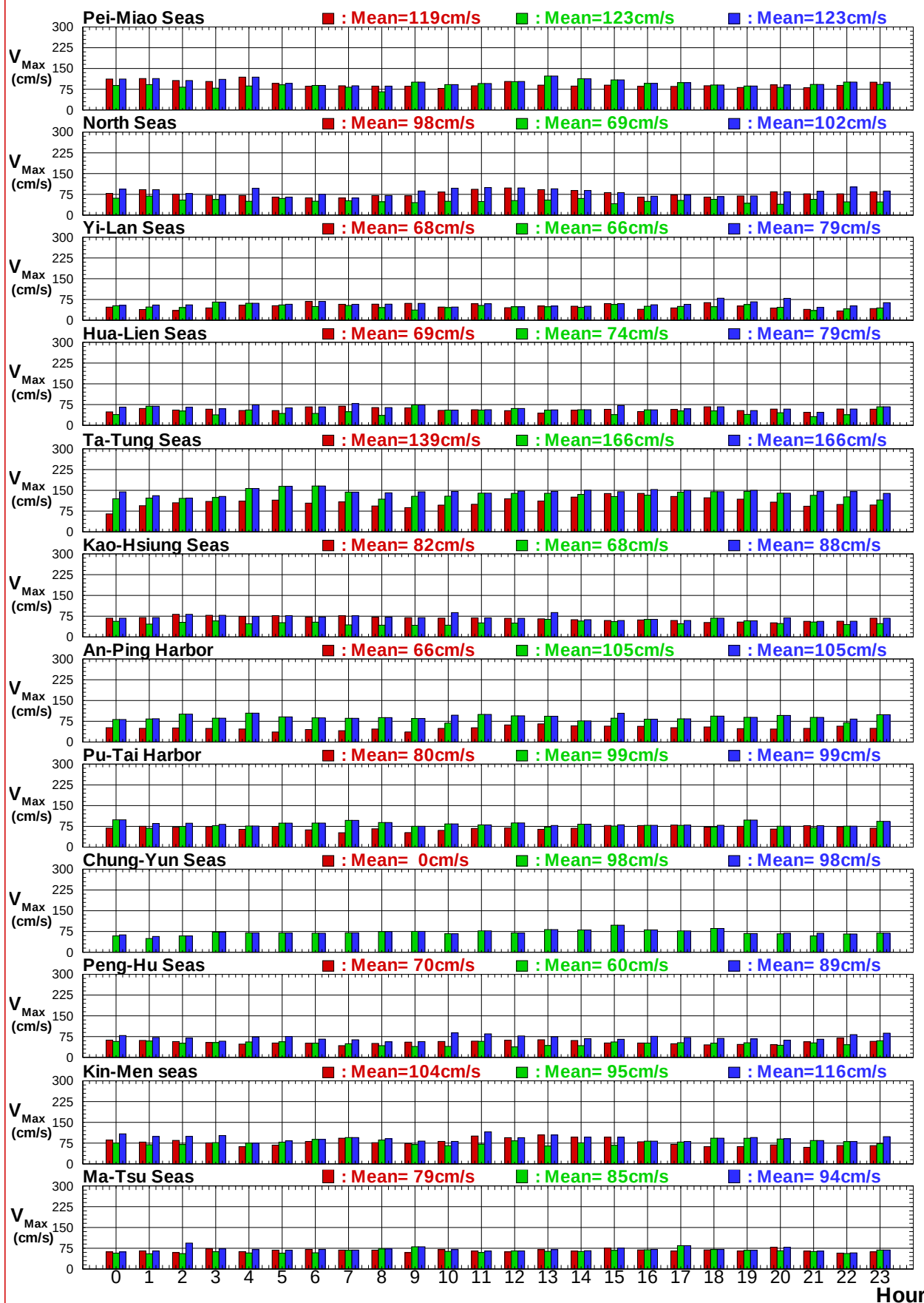
圖7.4c 2017年12港域冬、夏及整年主要測站逐時最大流速比較圖
