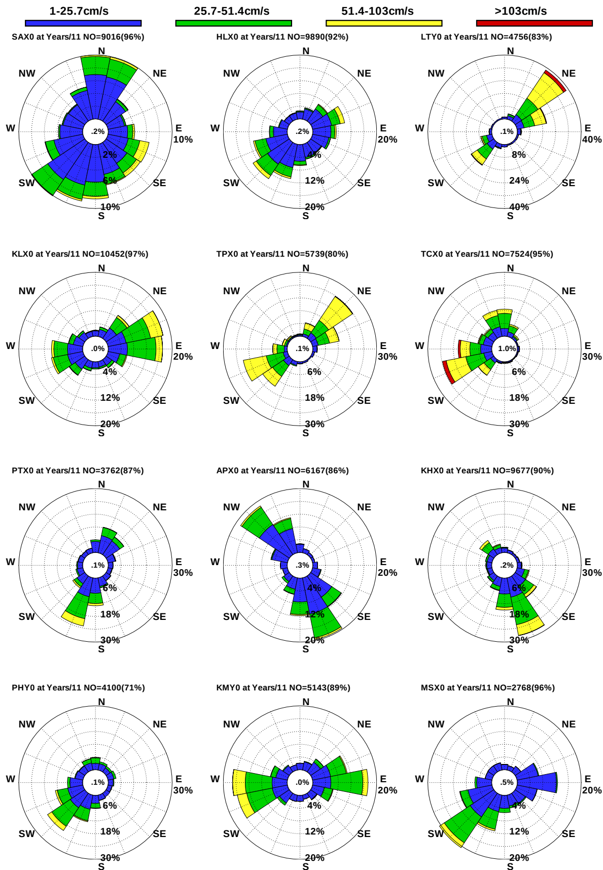
圖9.24 12港域歷年11月觀測海流玫瑰比較圖
