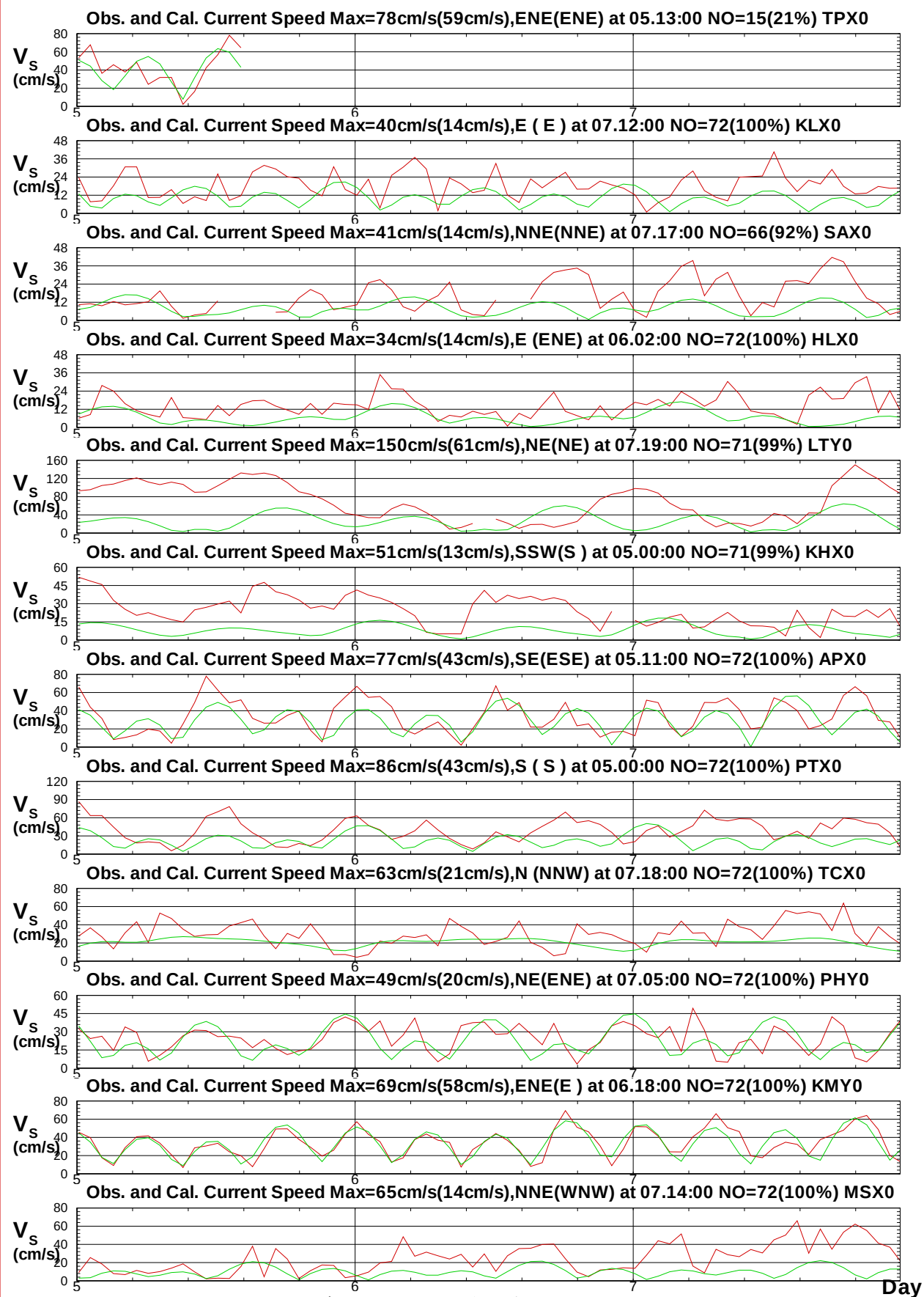
圖10.7 2017年谷超 颱風12海域觀測流速歷線圖 (綠色: 潮流)
