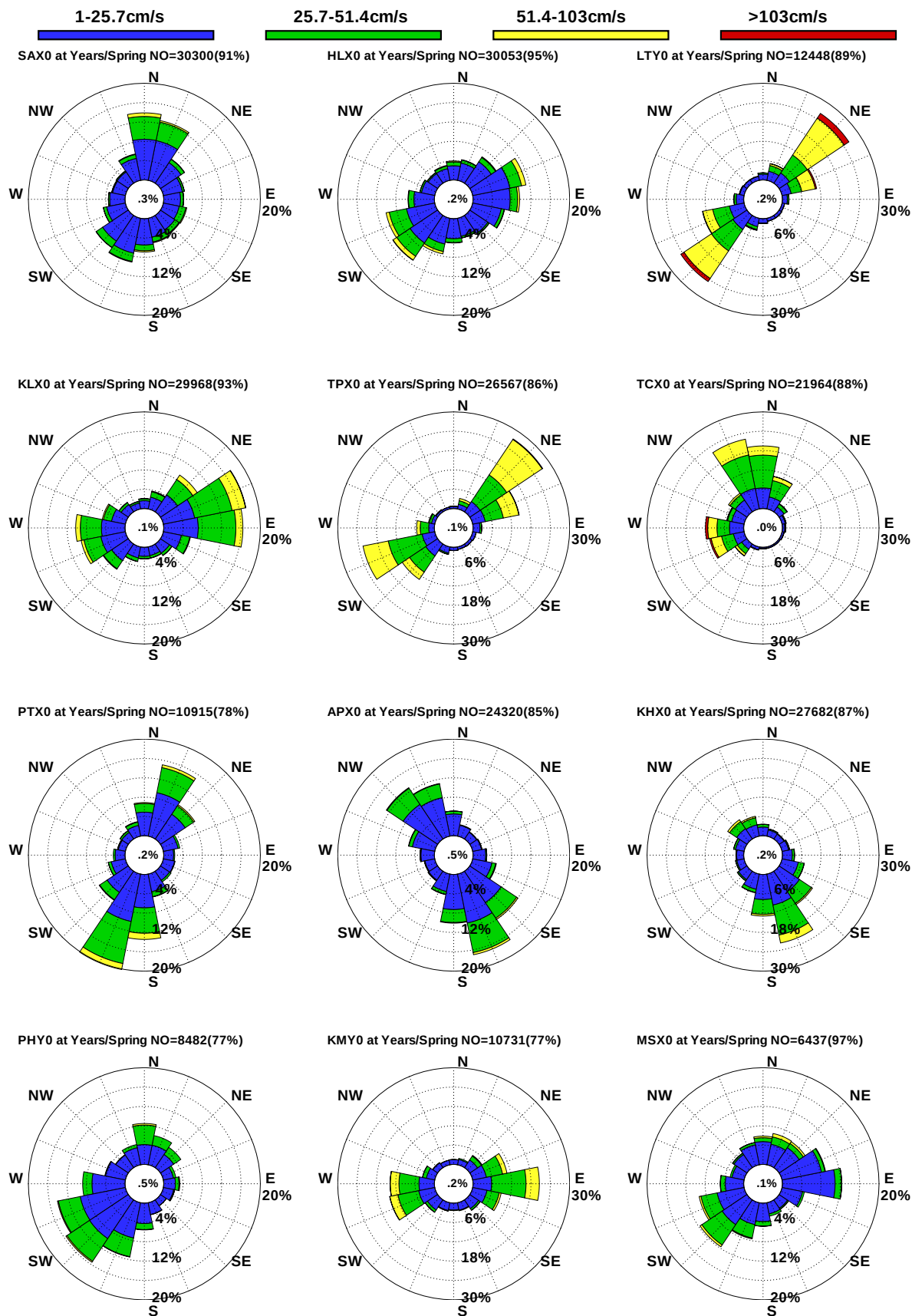
圖9.28 12港域歷年春季觀測海流玫瑰比較圖
