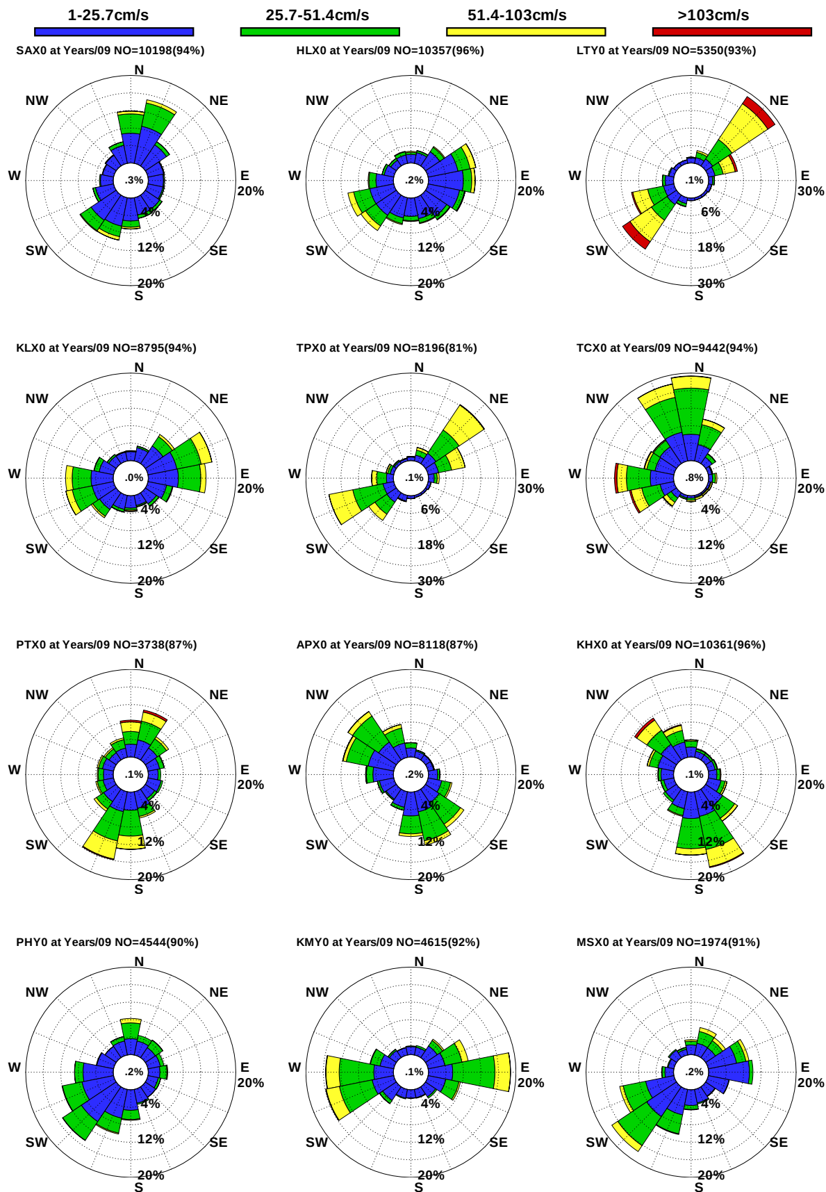
圖9.20 12港域歷年 9 月觀測海流玫瑰比較圖
