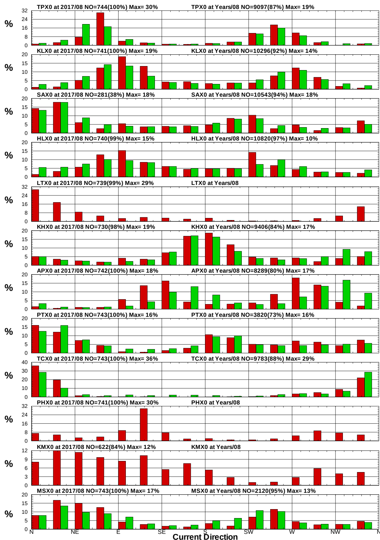
圖8.18 12港域2017年及歷年 8月流向統計方塊圖
