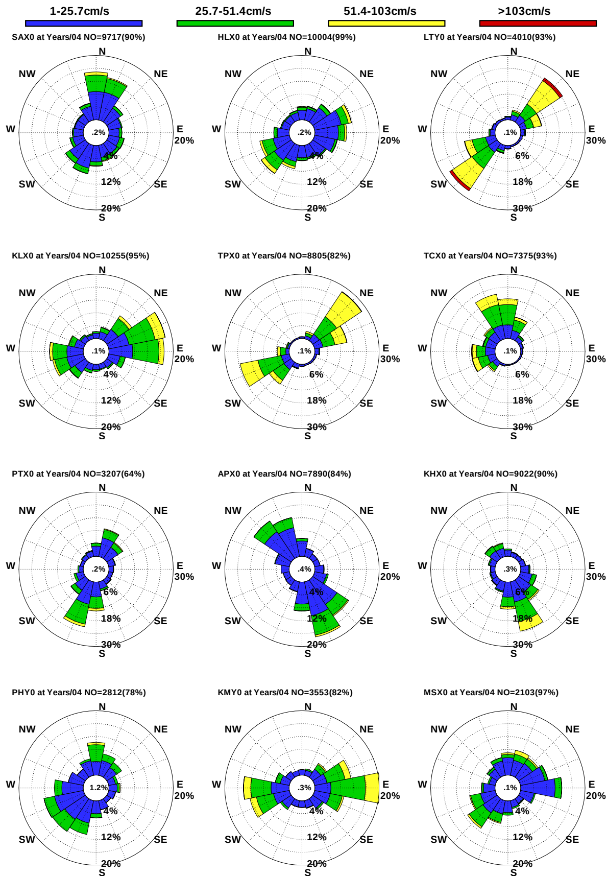
圖9.10 12港域歷年 4 月觀測海流玫瑰比較圖
