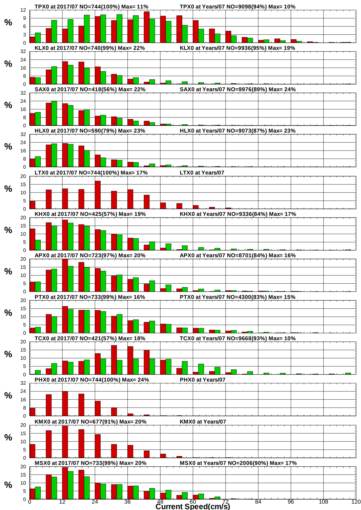
圖8.15 12港域2017年及歷年 7月流速統計方塊圖
