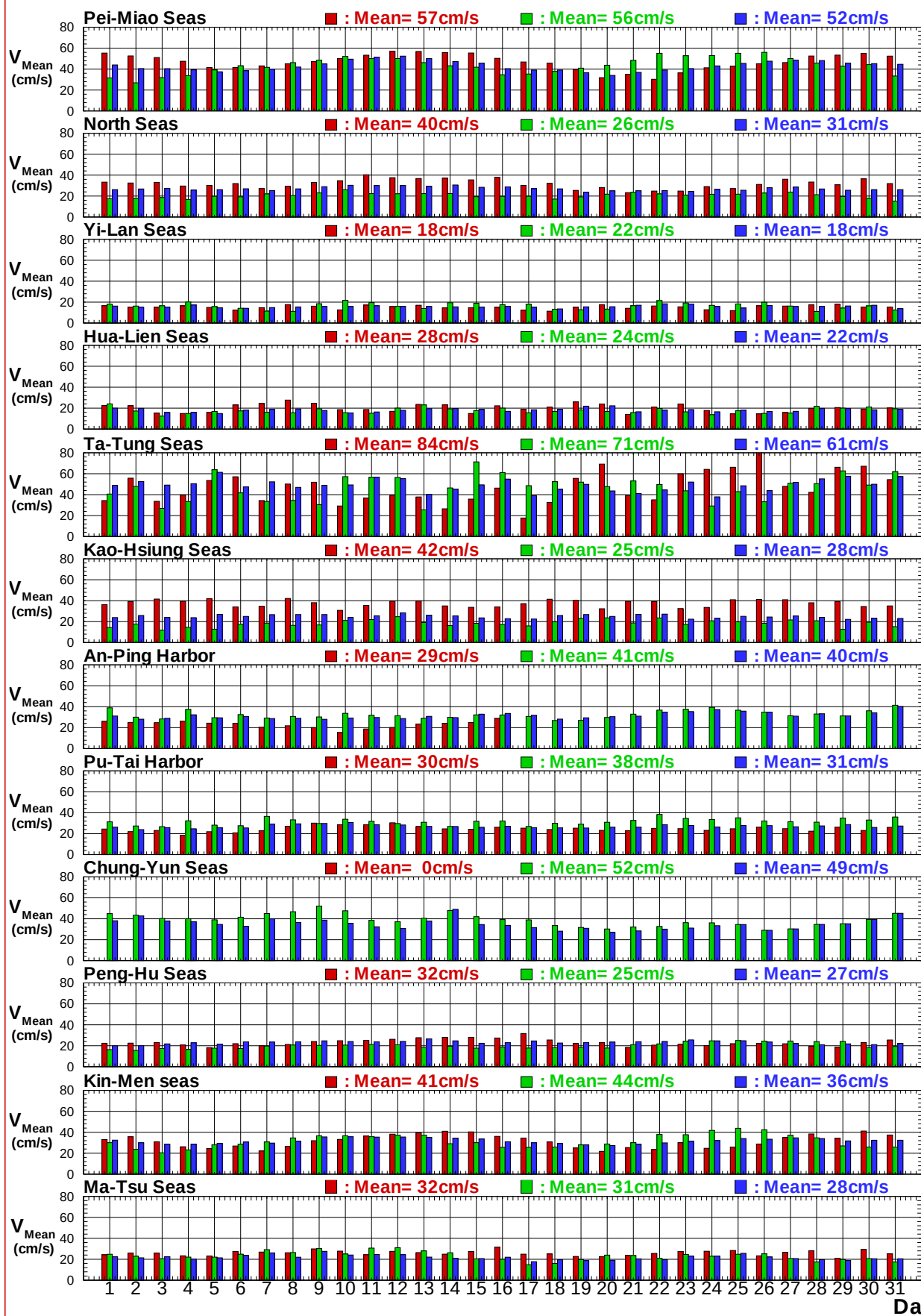
圖7.6a 2017年12港域冬, 夏及整年主要測站每日平均流速比較圖
