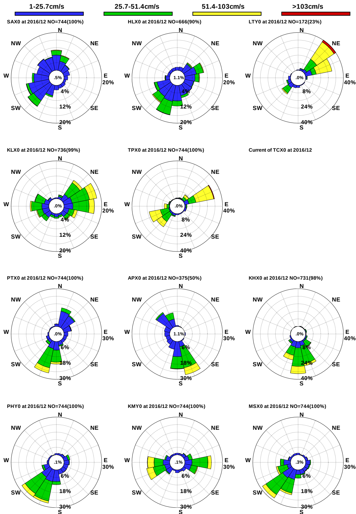
圖9.1 12港域2016年12月觀測海流玫瑰比較圖
