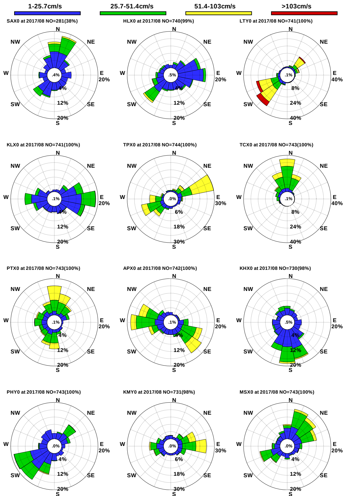
圖9.17 12港域2017年 8月觀測海流玫瑰比較圖
