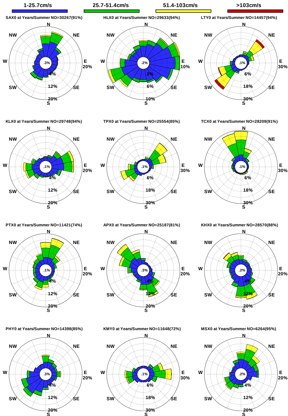
圖9.30 12港域歷年夏季觀測海流玫瑰比較圖
