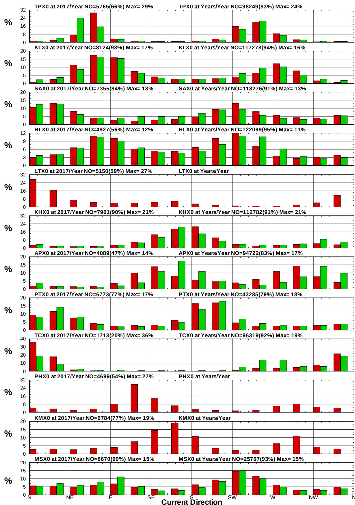
圖8.34 12港域2017年及歷年整年流向統計方塊圖
