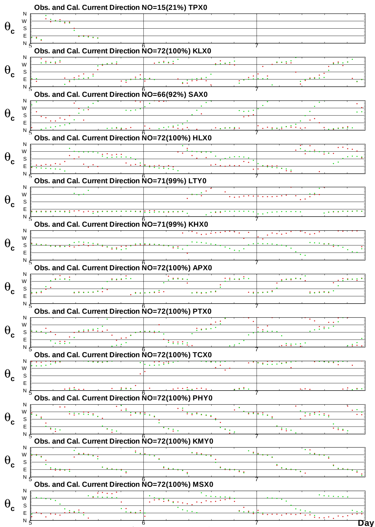
圖10.8 2017年谷超 颱風12海域觀測流向歷線圖 (綠色: 潮流)
