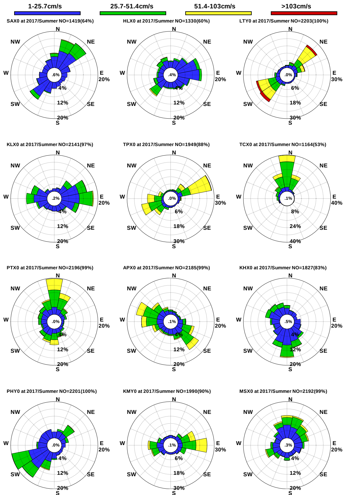
圖9.29 12港域2017年夏季觀測海流玫瑰比較圖
