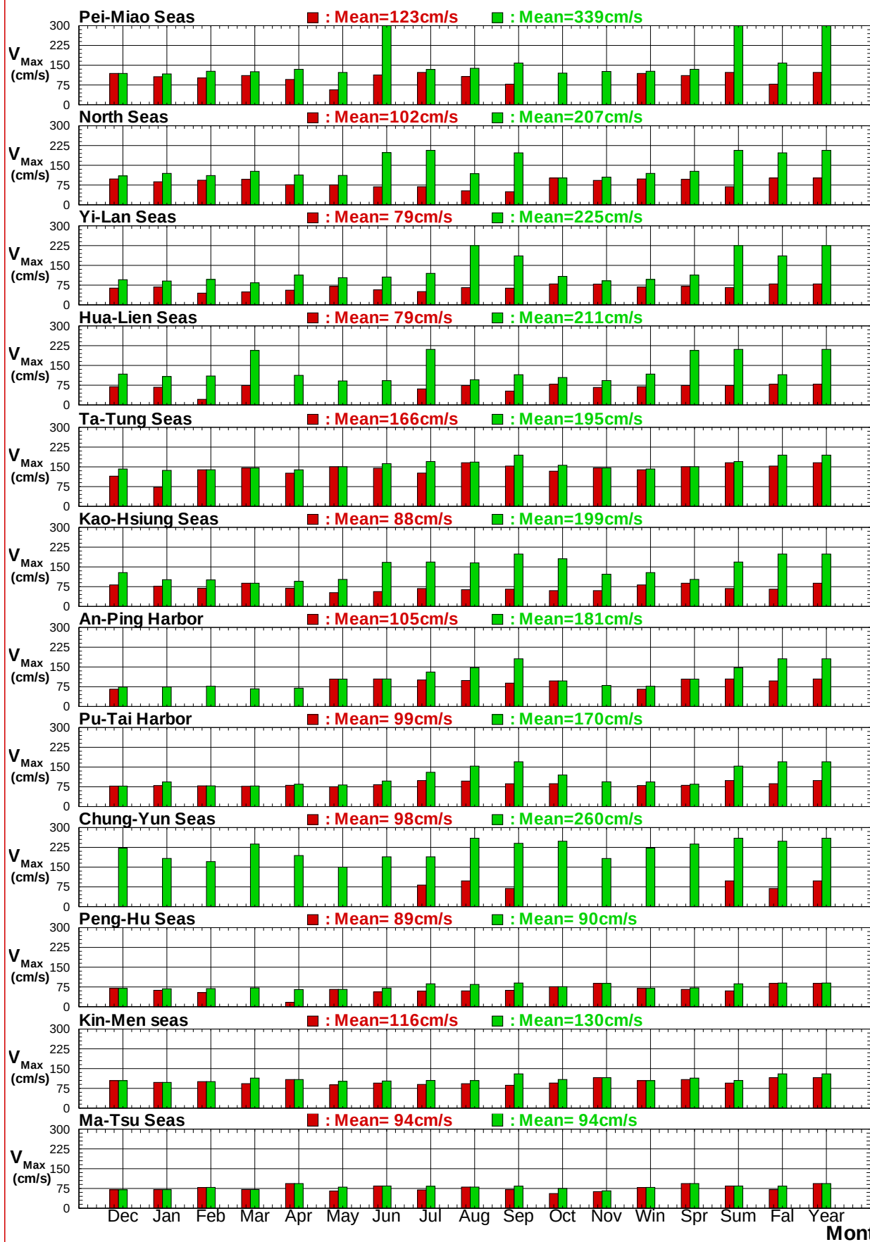
圖7.3c 2017及歷年12港域主要測站每月(季)最大流速比較圖
