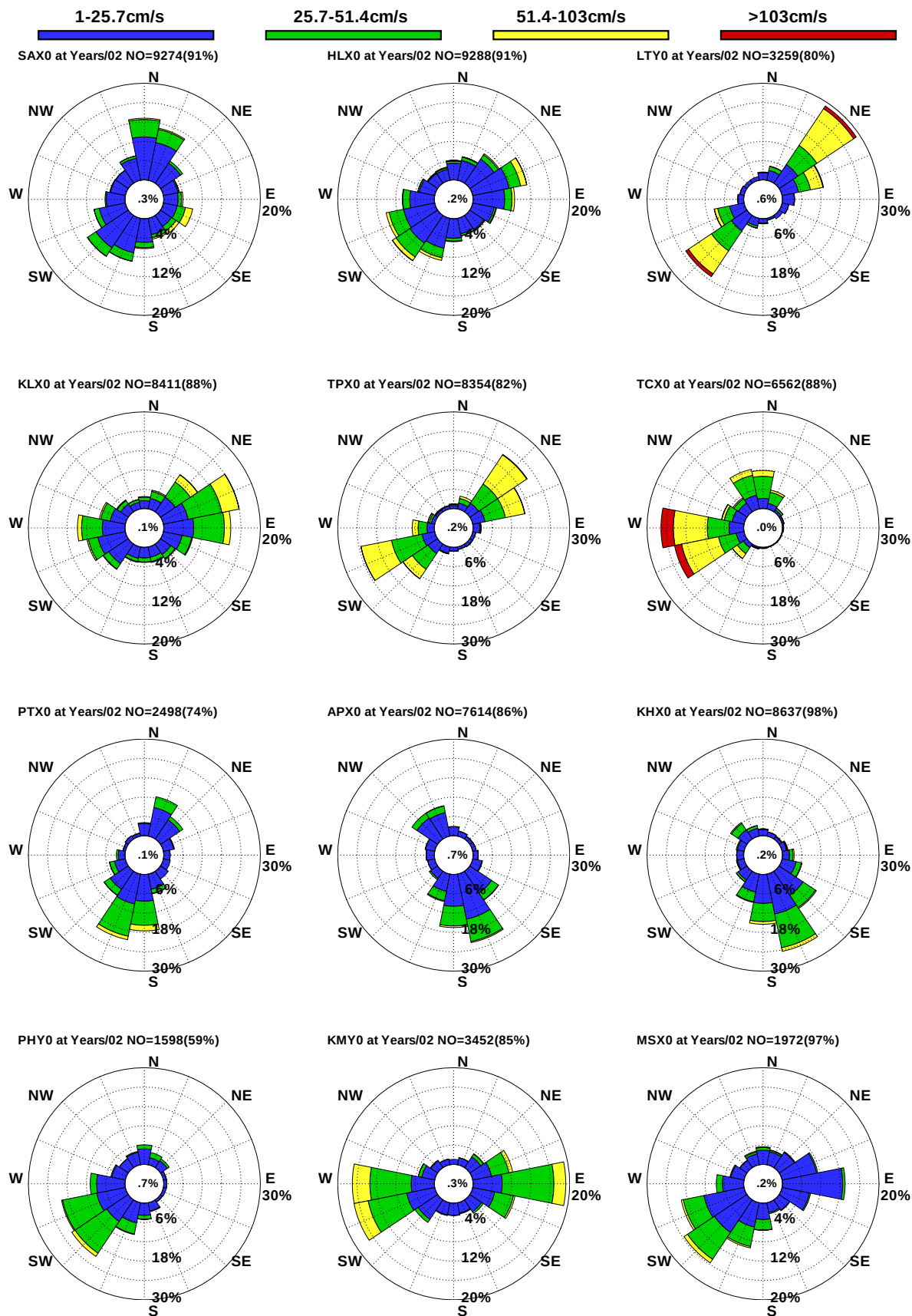
圖9.6 12港域歷年 2 月觀測海流玫瑰比較圖
