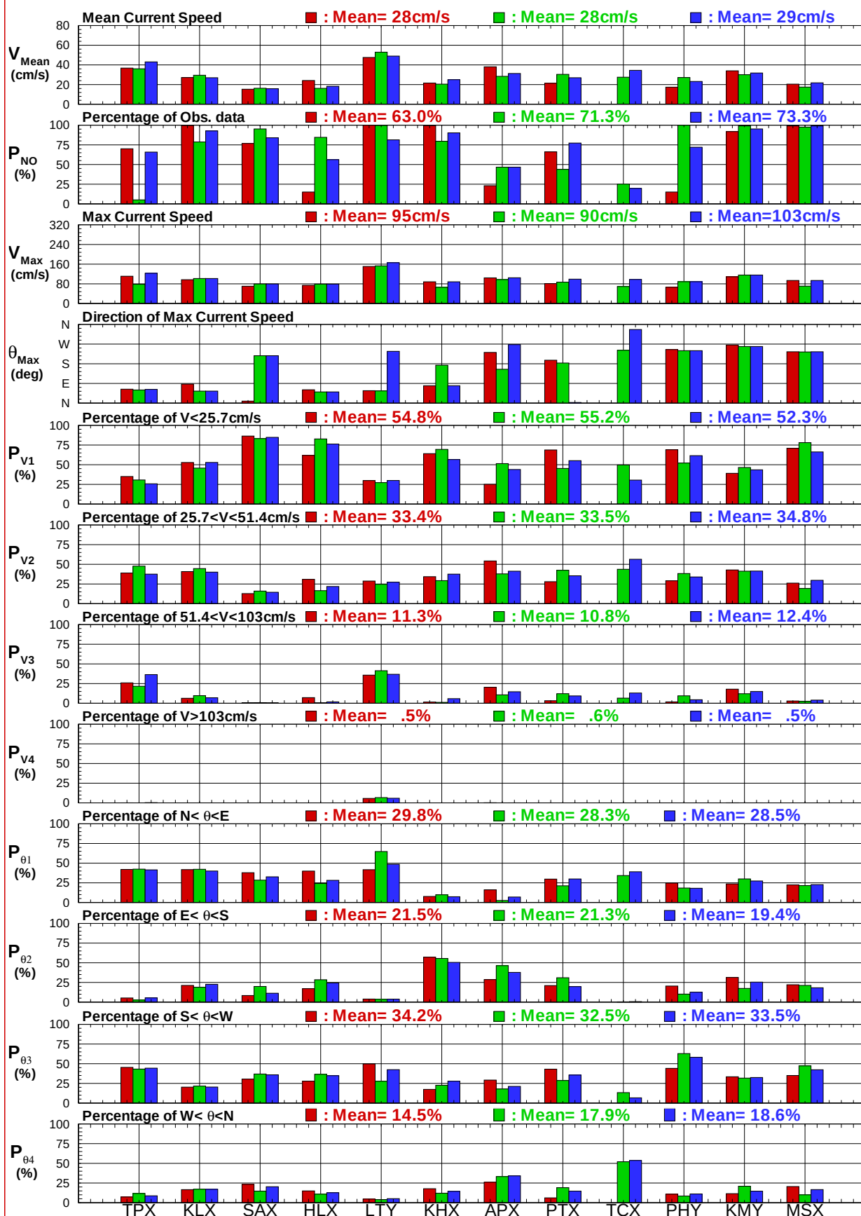
圖7.2c 12個港域2017年主要測站春、秋及整年流速 (向) 比較圖
