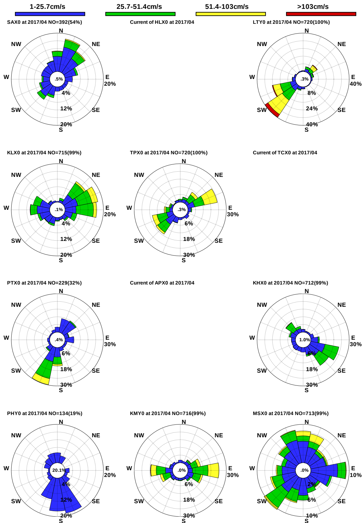
圖9.9 12港域2017年 4月觀測海流玫瑰比較圖
