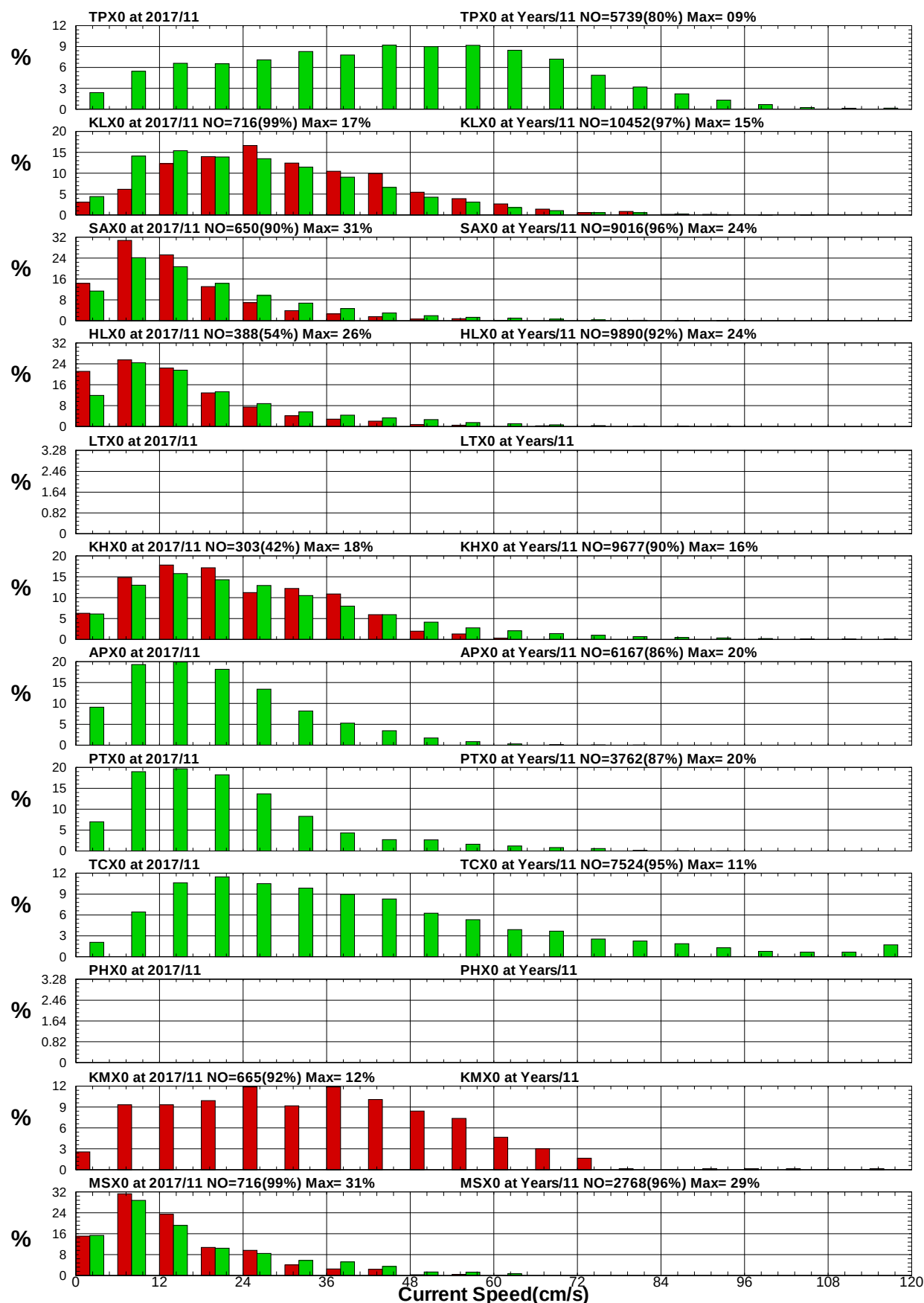
圖8.23 12港域2017年及歷年11月流速統計方塊圖
