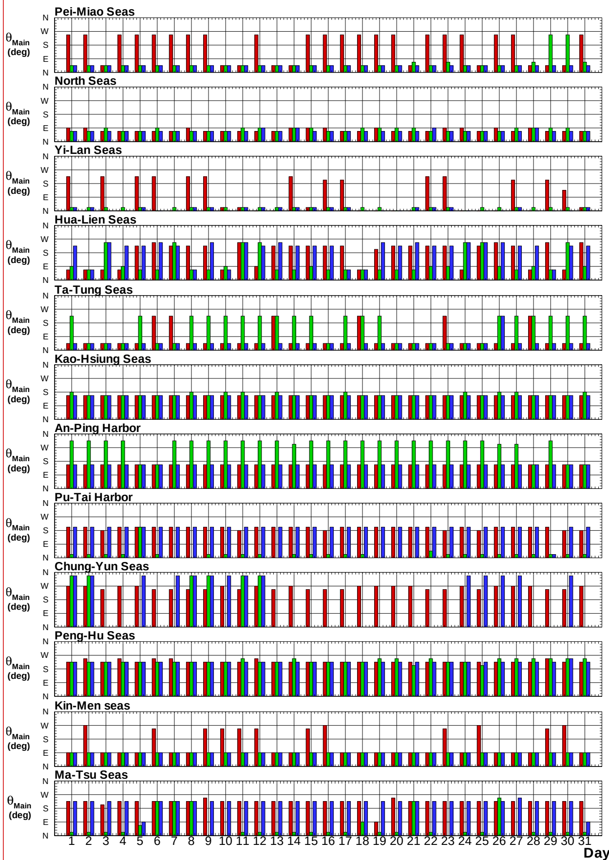
圖7.7e 歷年12港域冬, 夏及整年主要測站每日主要流向比較圖
