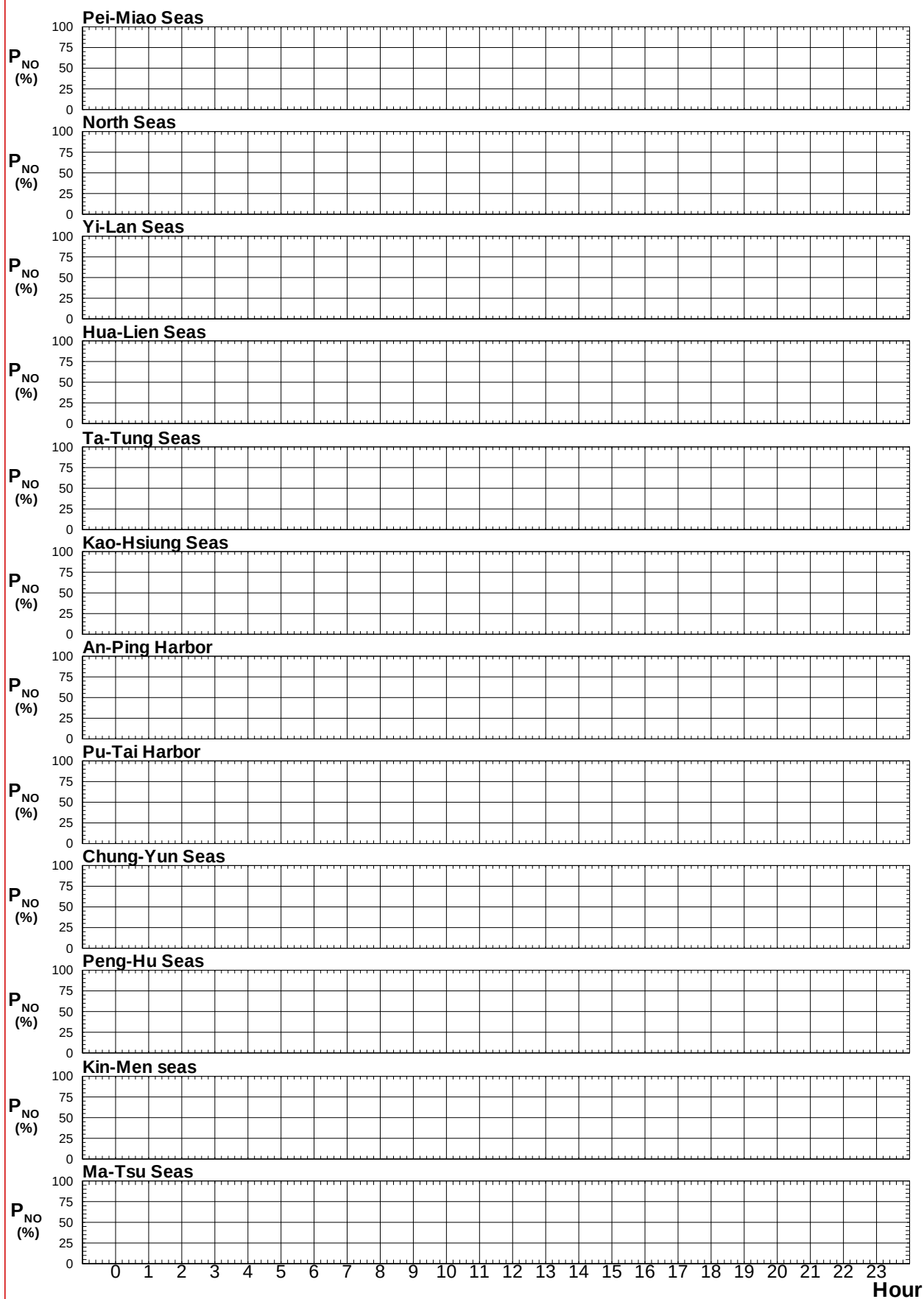
圖7.5b 歷年12港域冬, 夏及整年主要測站逐時蒐集率比較圖
