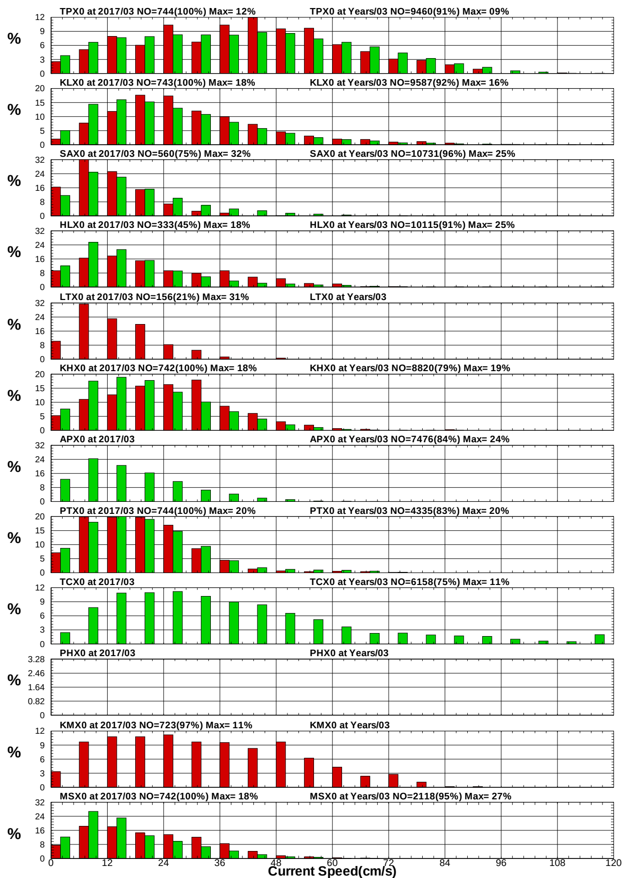
圖8.7 12港域2017年及歷年 3月流速統計方塊圖
