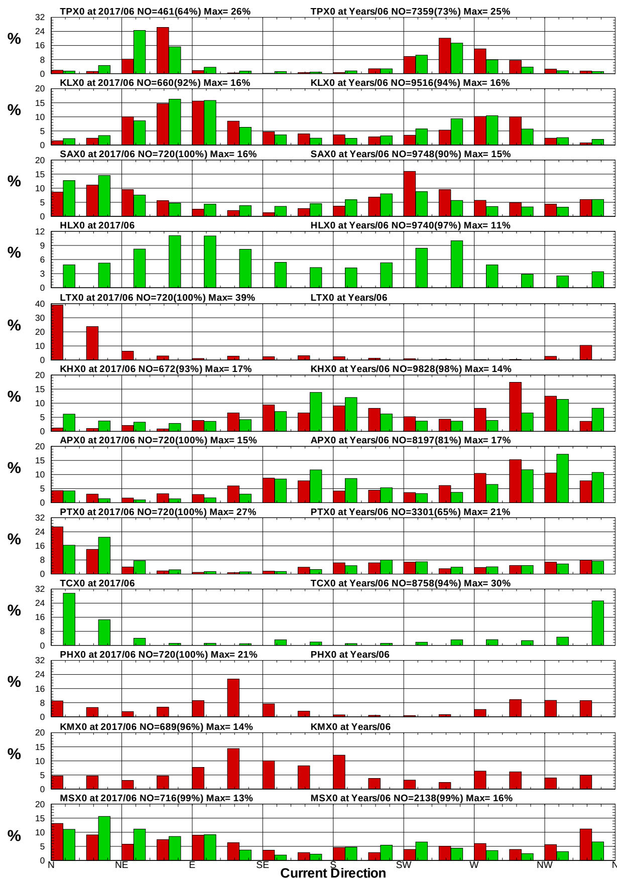
圖8.14 12港域2017年及歷年 6月流向統計方塊圖
