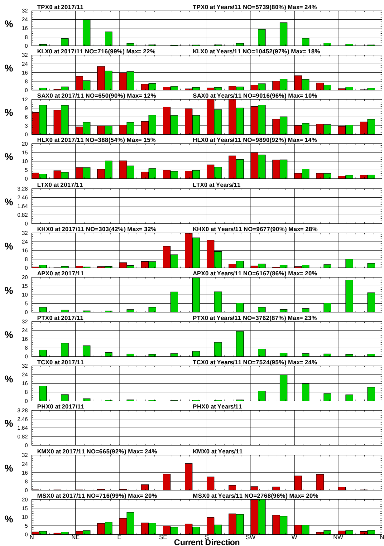
圖8.24 12港域2017年及歷年11月流向統計方塊圖
