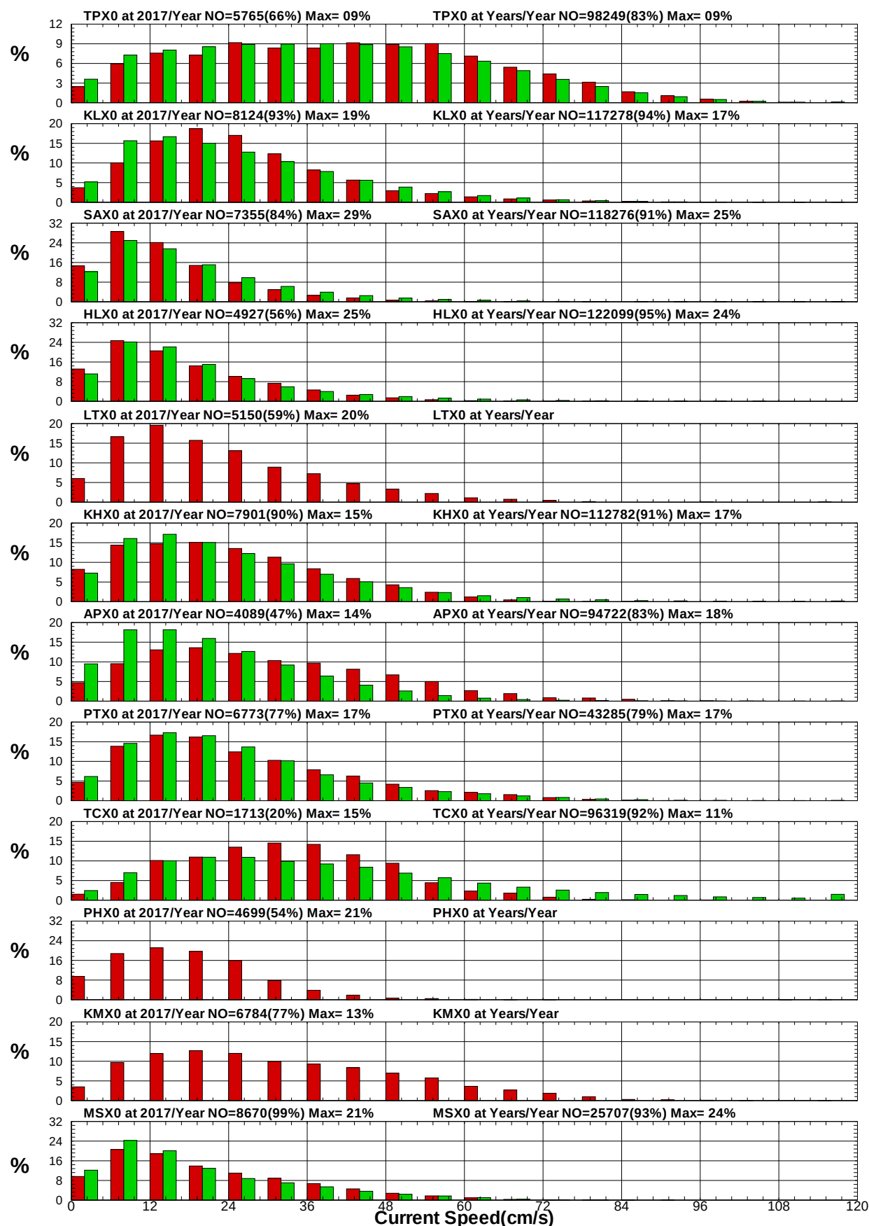
圖8.33 12港域2017年及歷年整年流速統計方塊圖
