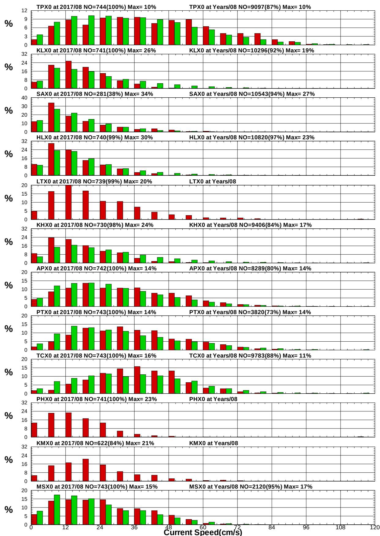
圖8.17 12港域2017年及歷年 8月流速統計方塊圖
