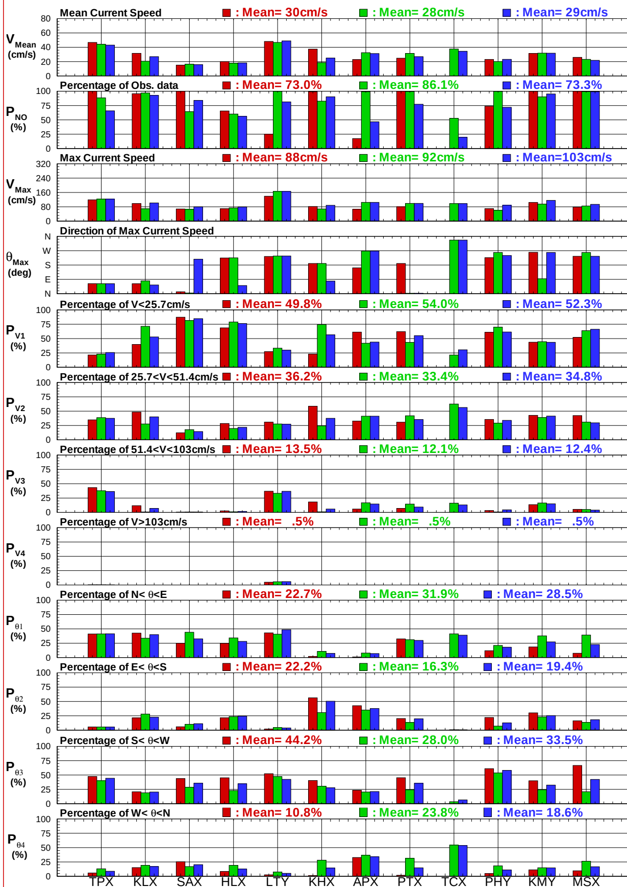
圖7.2a 12個港域2017年主要測站冬, 夏及整年流速 (向) 比較圖
