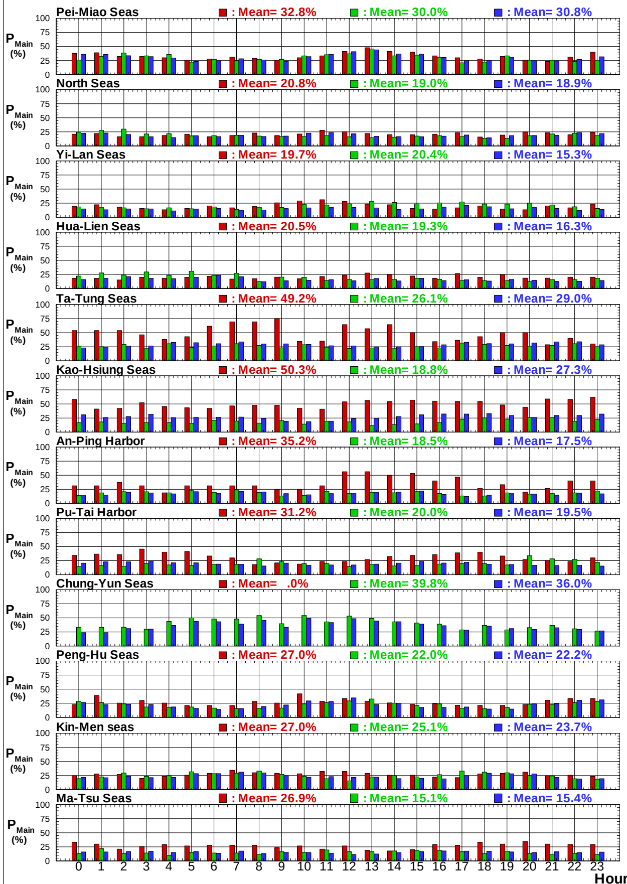
圖7.4f 2017年12港域冬, 夏及整年主要測站逐時主要流向百分比圖
