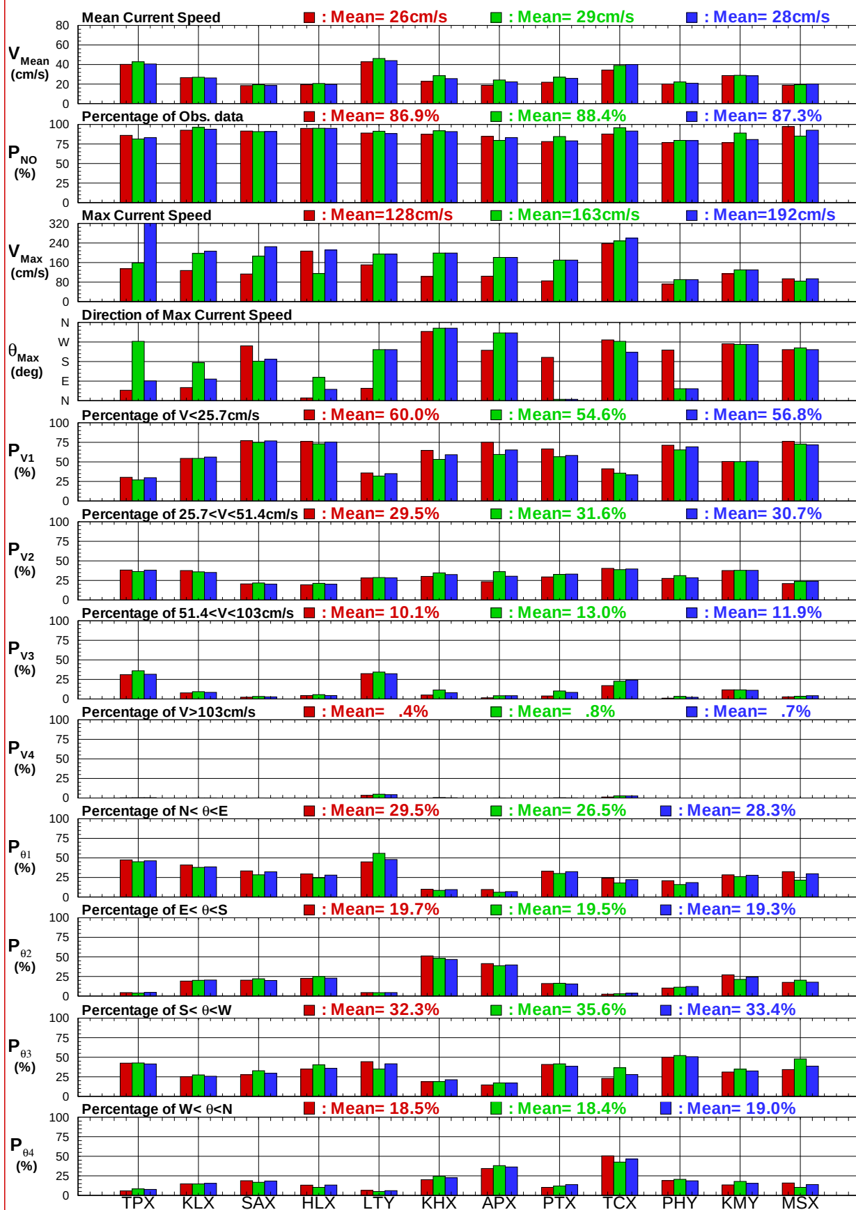
圖7.2d 12個港域歷年主要測站春, 秋及整年流速 (向) 比較圖
