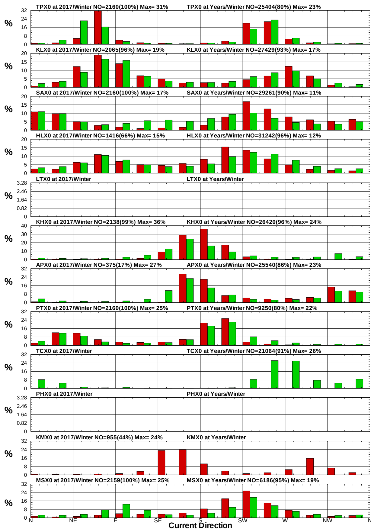
圖8.26 12港域2017年及歷年冬季流向統計方塊圖
