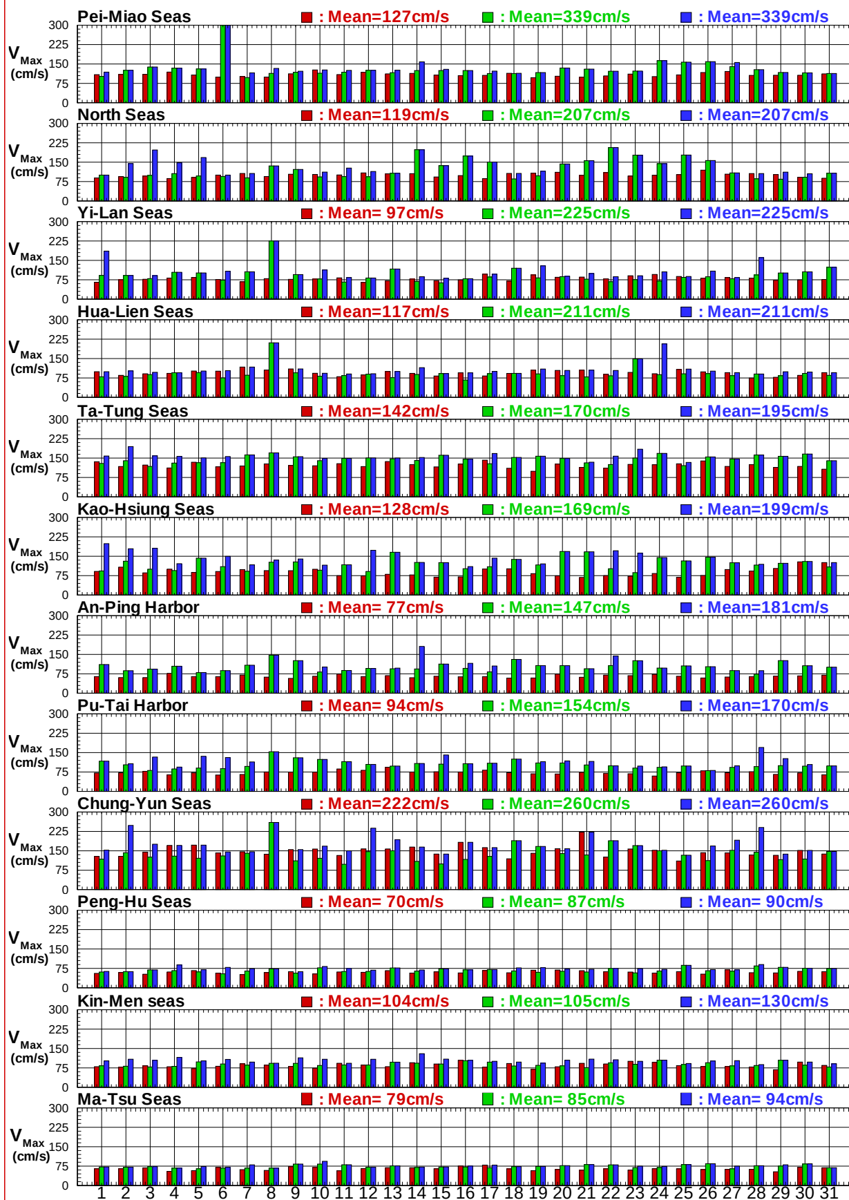
圖7.7c 歷年12港域冬, 夏及整年主要測站每日最大流速比較圖
