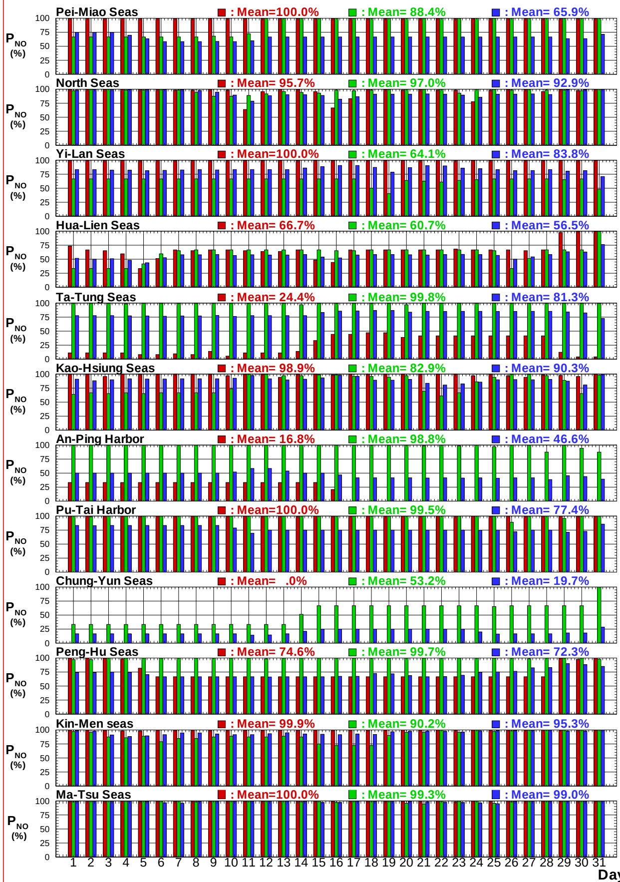
圖7.6b 2017年12港域冬, 夏及整年主要測站每日蒐集率比較圖
