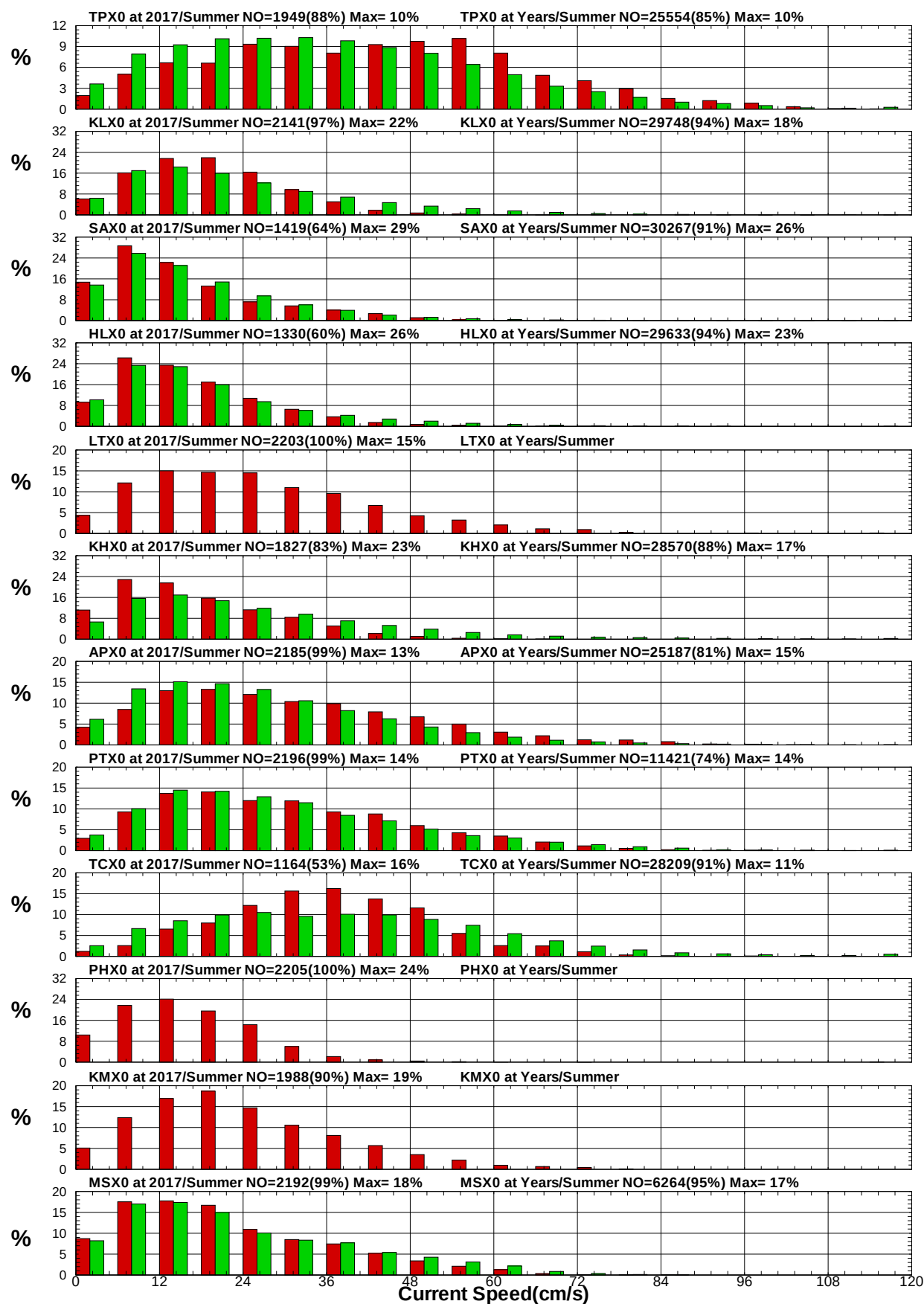
圖8.29 12港域2017年及歷年夏季流速統計方塊圖
