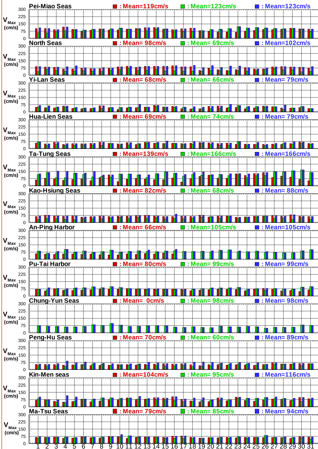
圖7.6c 2017年12港域冬、夏及整年主要測站每日最大流速比較圖
