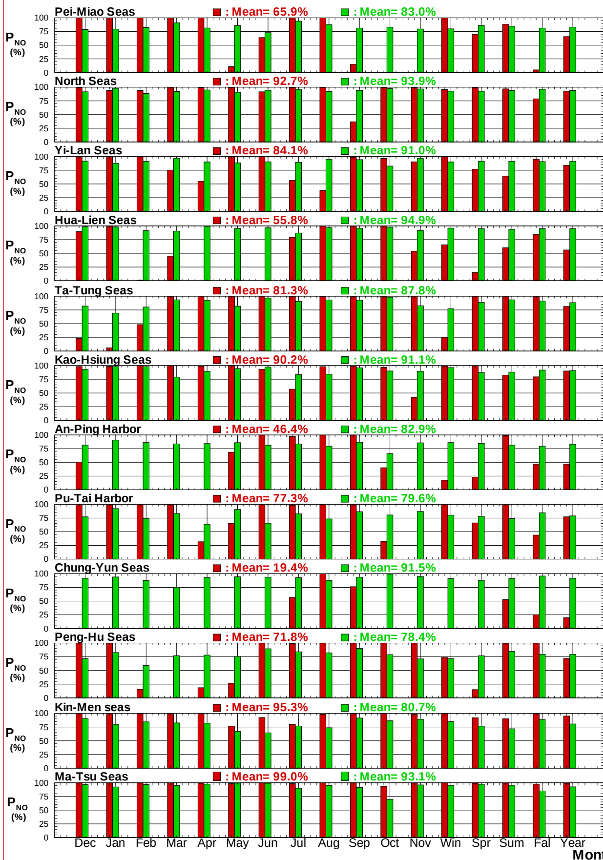
圖7.3b 2017及歷年12港域主要測站每月(季)蒐集率比較圖
