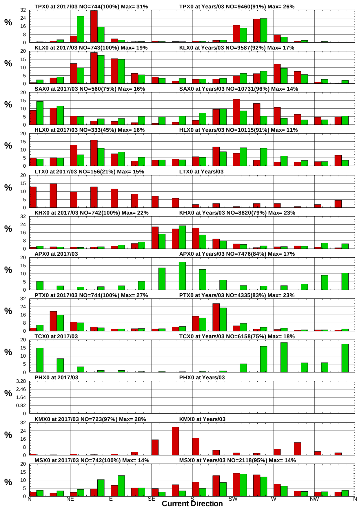
圖8.8 12港域2017年及歷年 3月流向統計方塊圖
