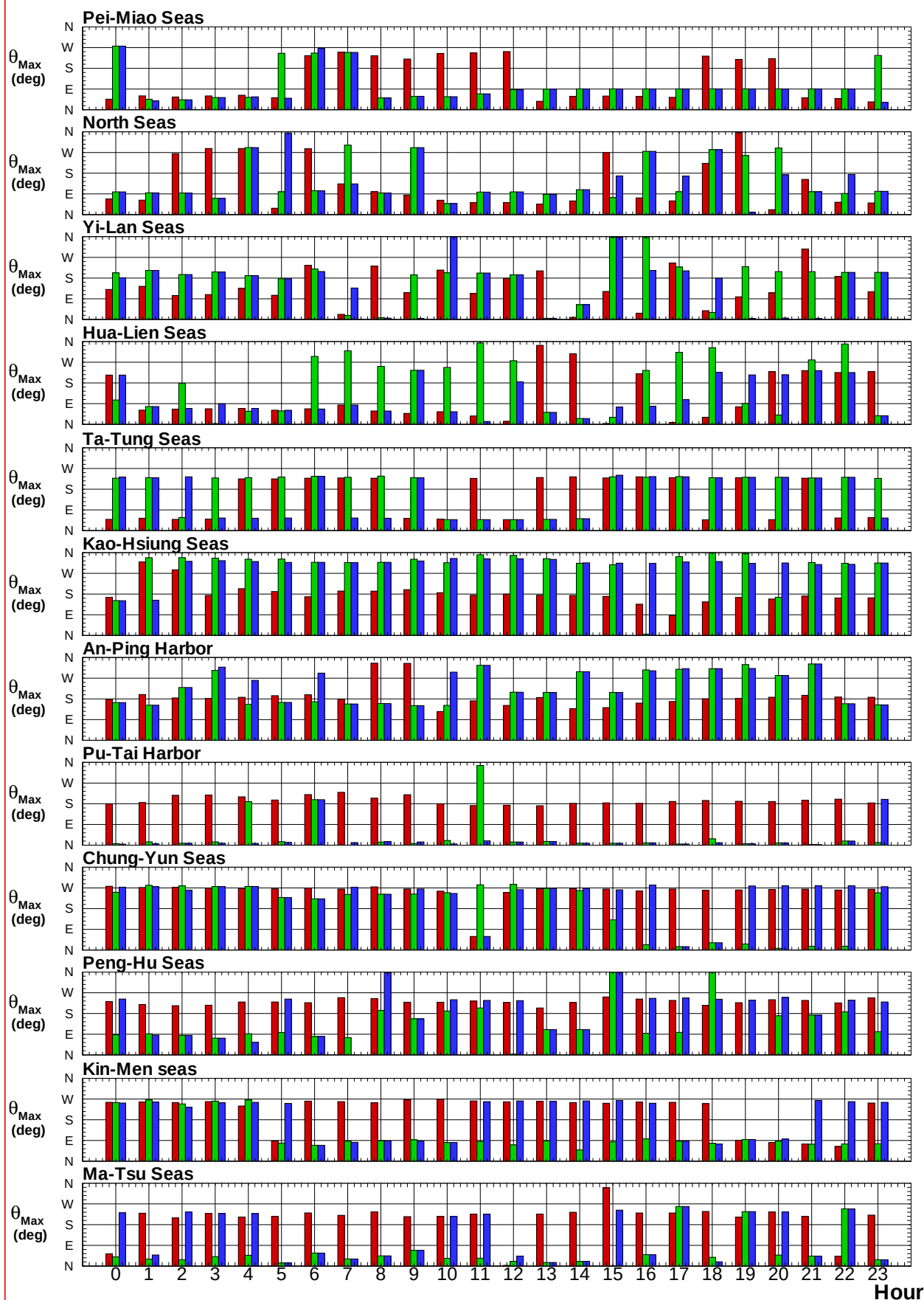
圖7.5d 歷年12港域冬, 夏及整年主要測站逐時最大流速之流向圖
