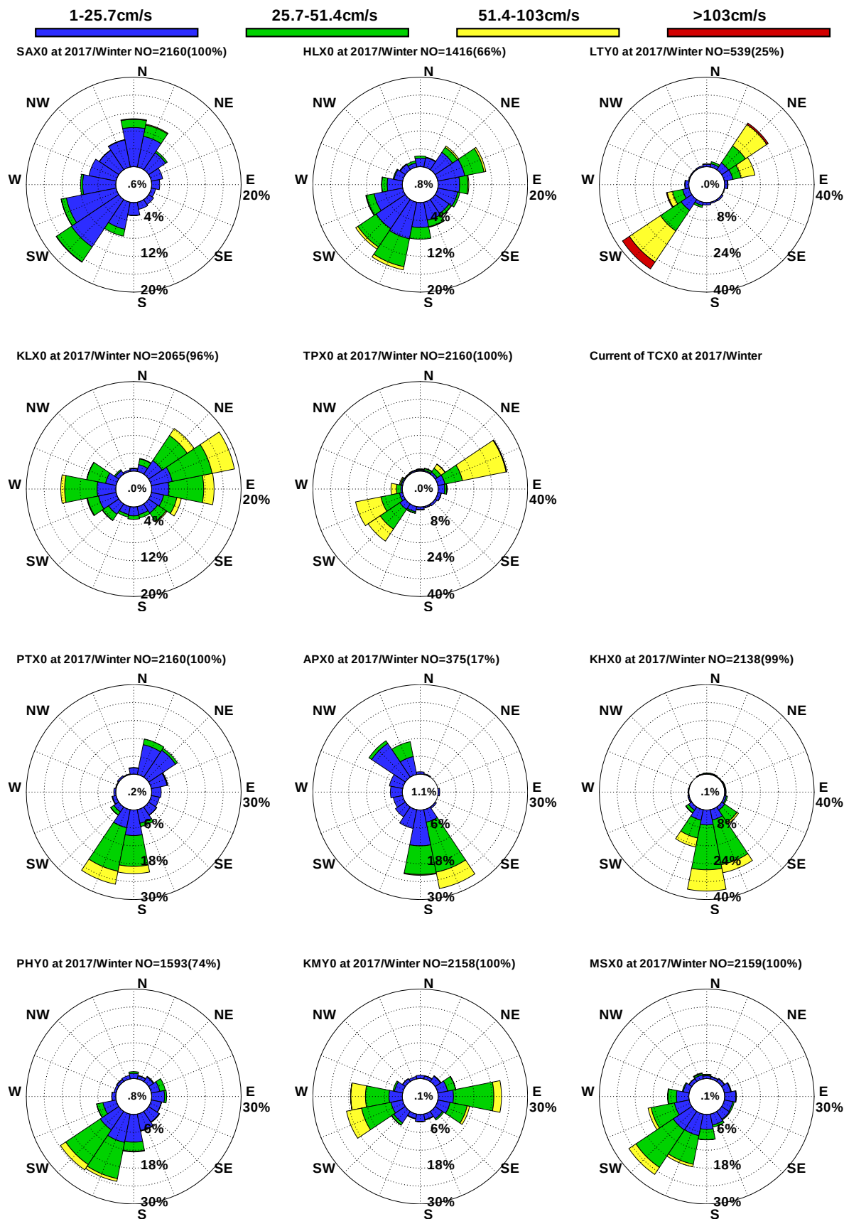
圖9.25 12港域2017年冬季觀測海流玫瑰比較圖
