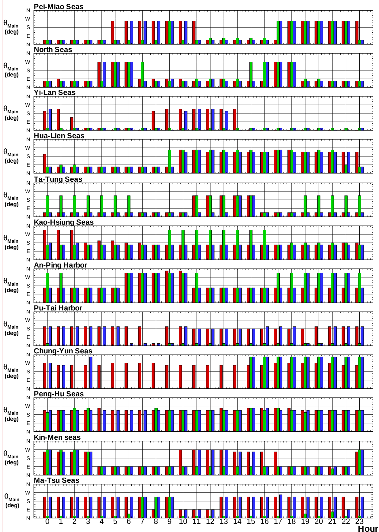
圖7.5e 歷年12港域冬, 夏及整年主要測站逐時主要流向比較圖
