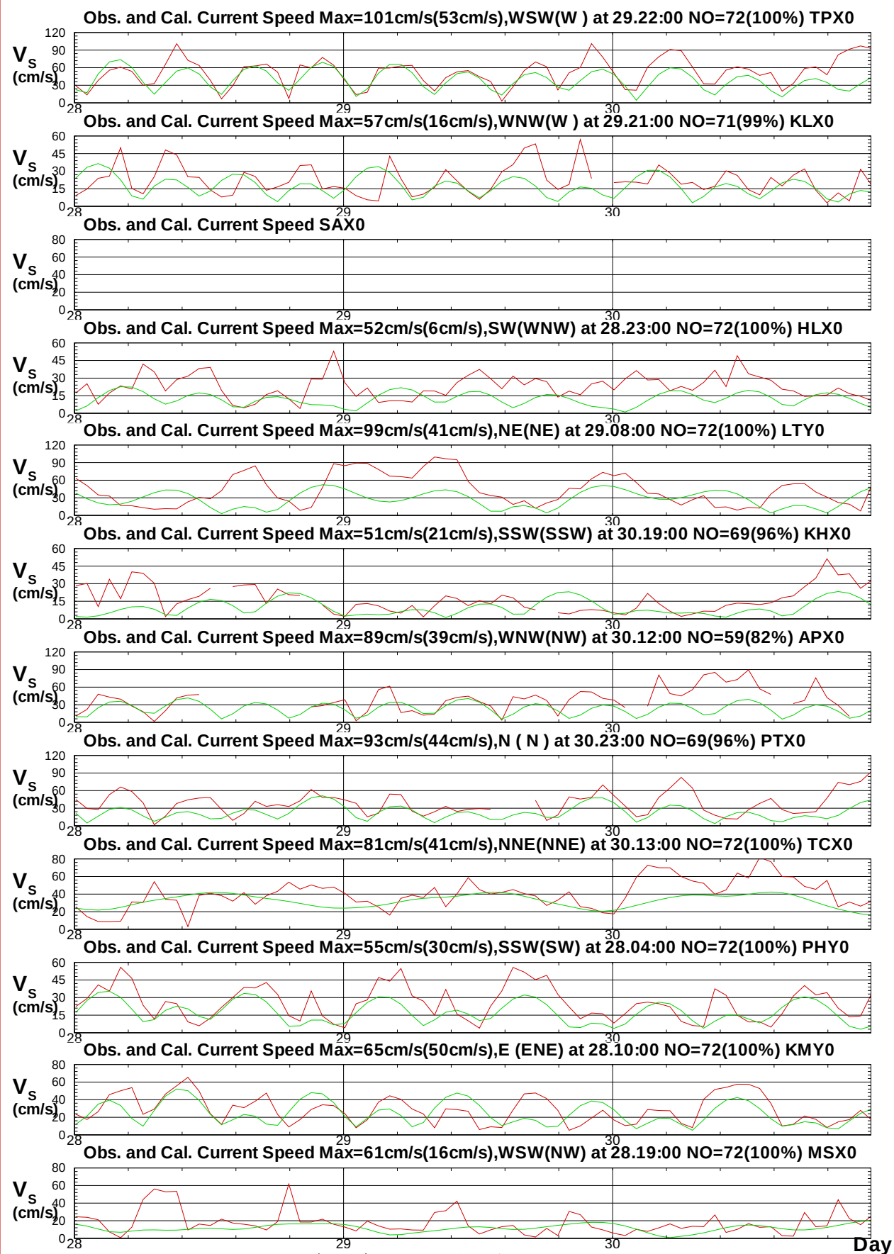
圖10.1 2017年尼莎 颱風12海域觀測流速歷線圖 (綠色: 潮流)
