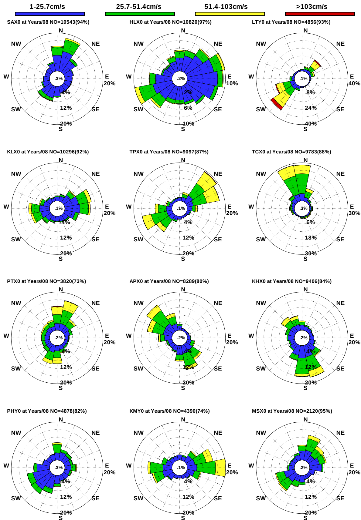
圖9.18 12港域歷年 8 月觀測海流玫瑰比較圖
