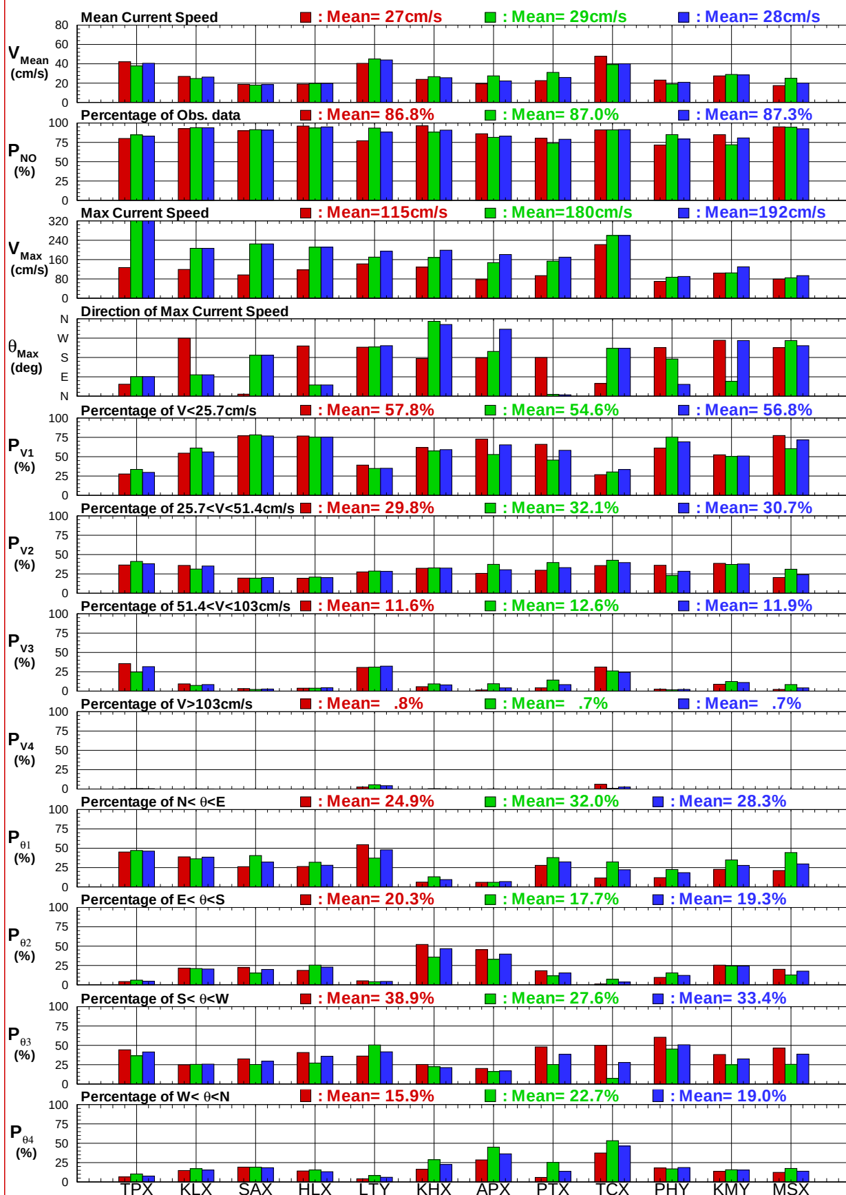
圖7.2b 12個港域歷年主要測站冬, 夏及整年流速 (向) 比較圖
