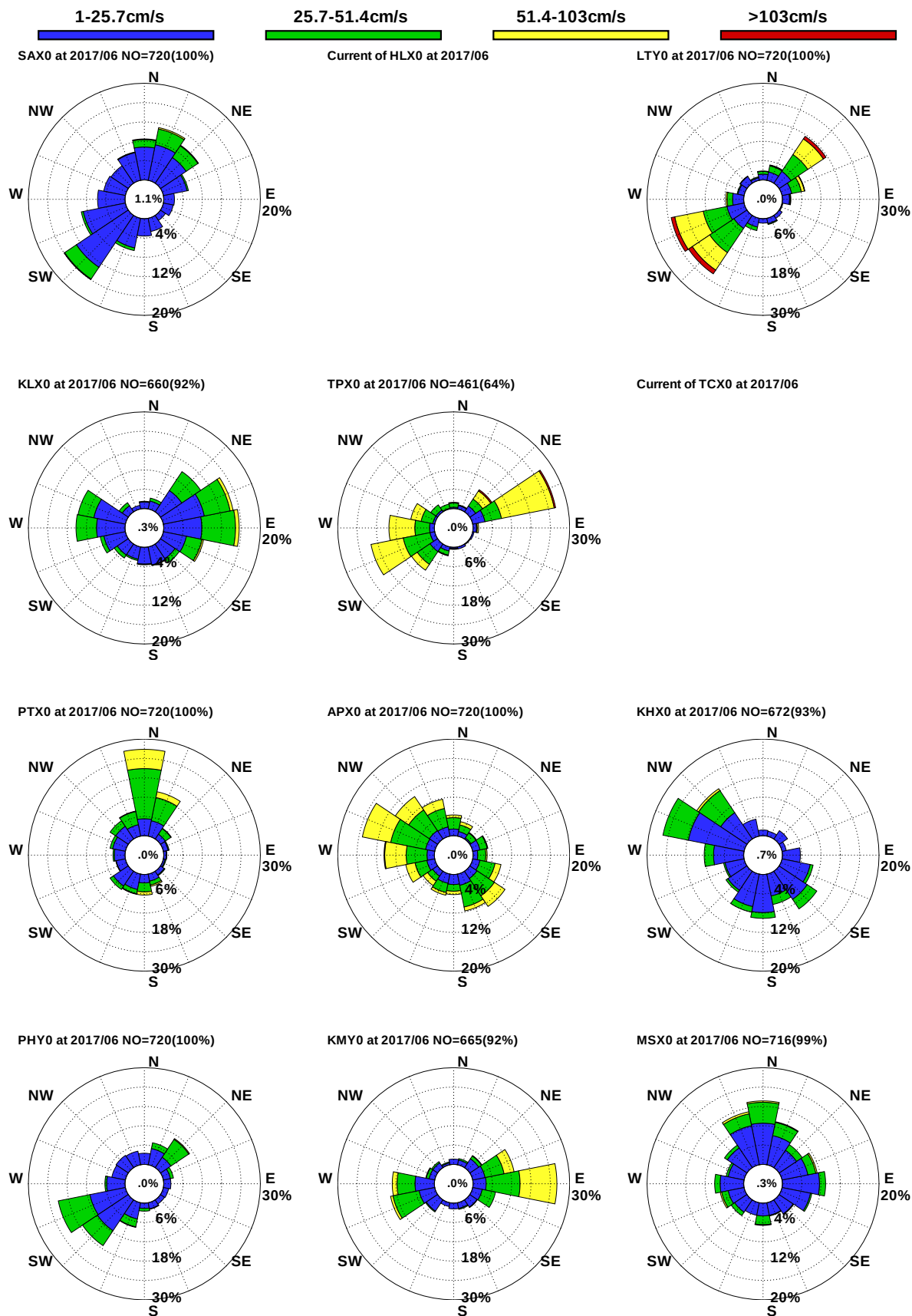
圖9.13 12港域2017年 6月觀測海流玫瑰比較圖
