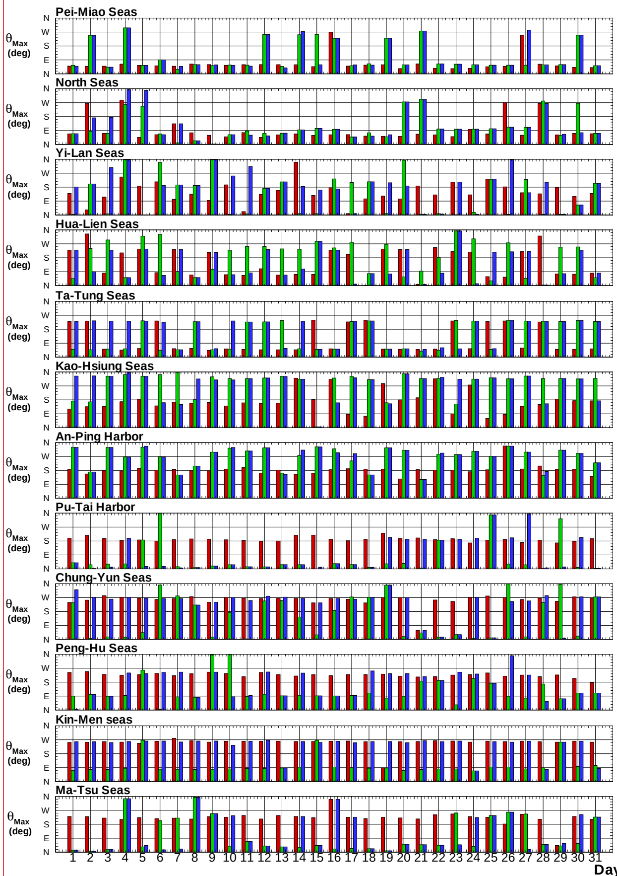
圖7.7d 歷年12港域冬, 夏及整年主要測站每日最大流速之流向圖
