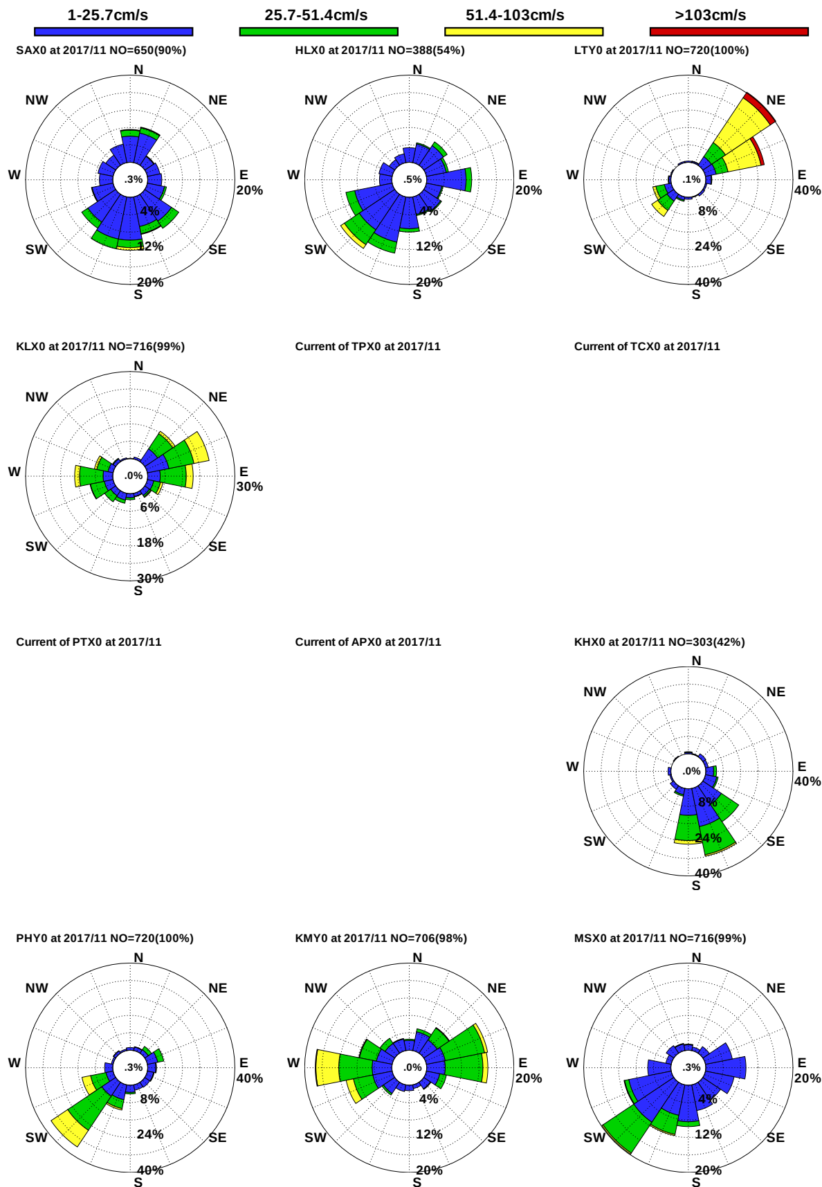
圖9.23 12港域2017年11月觀測海流玫瑰比較圖
