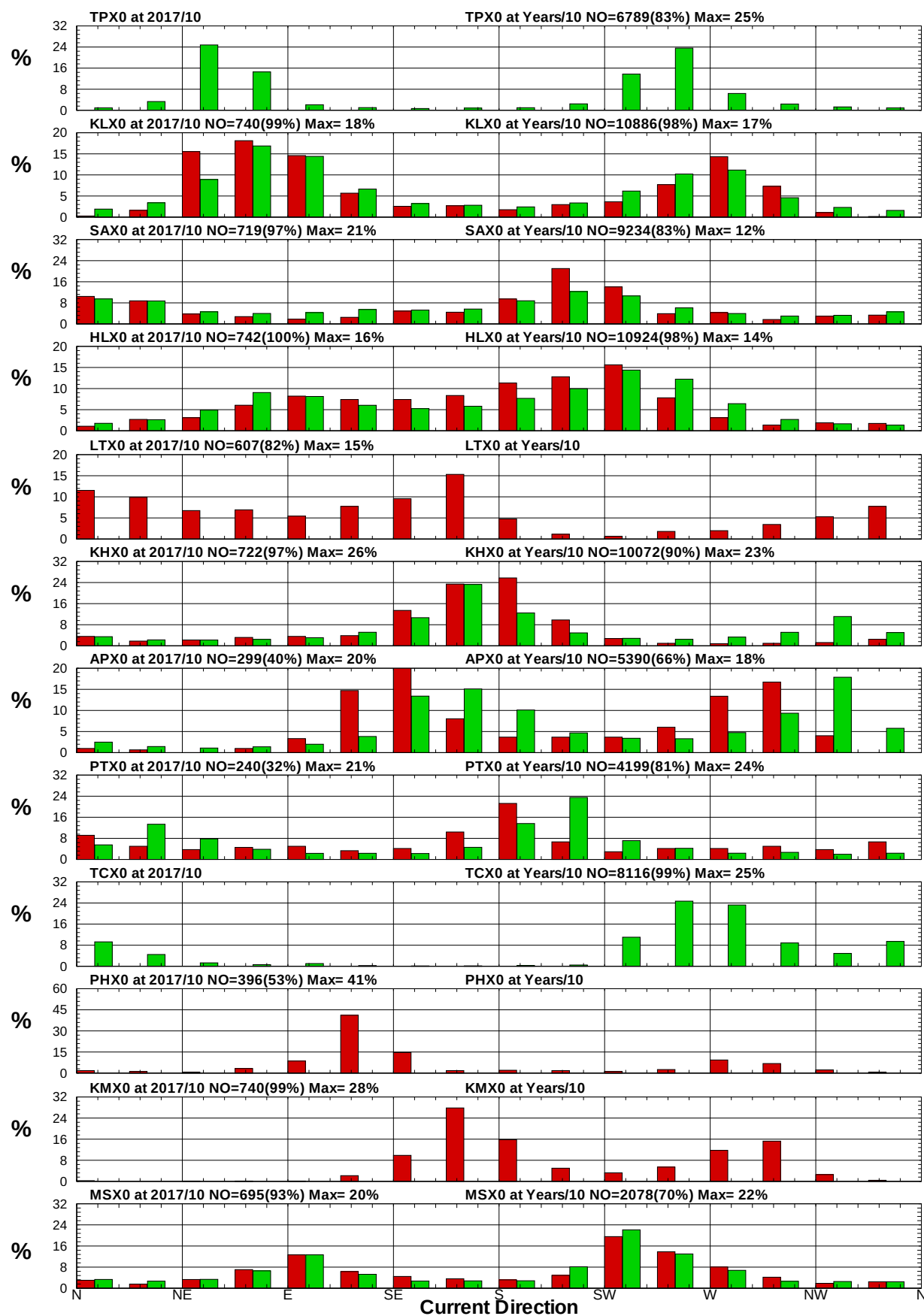
圖8.22 12港域2017年及歷年10月流向統計方塊圖
