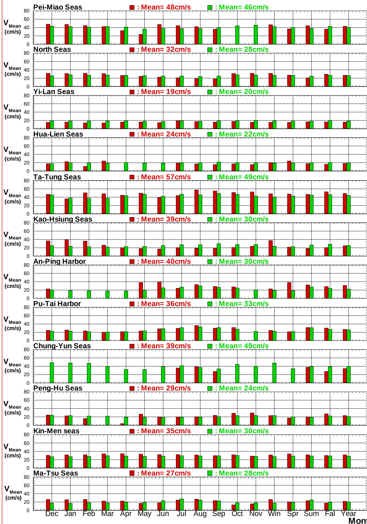
圖7.3a 2017及歷年12港域主要測站每月(季) 平均流速比較圖
