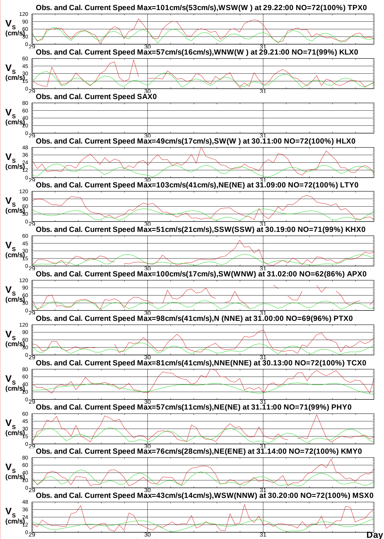
圖10.3 2017年海棠 颱風12海域觀測流速歷線圖 (綠色: 潮流)
