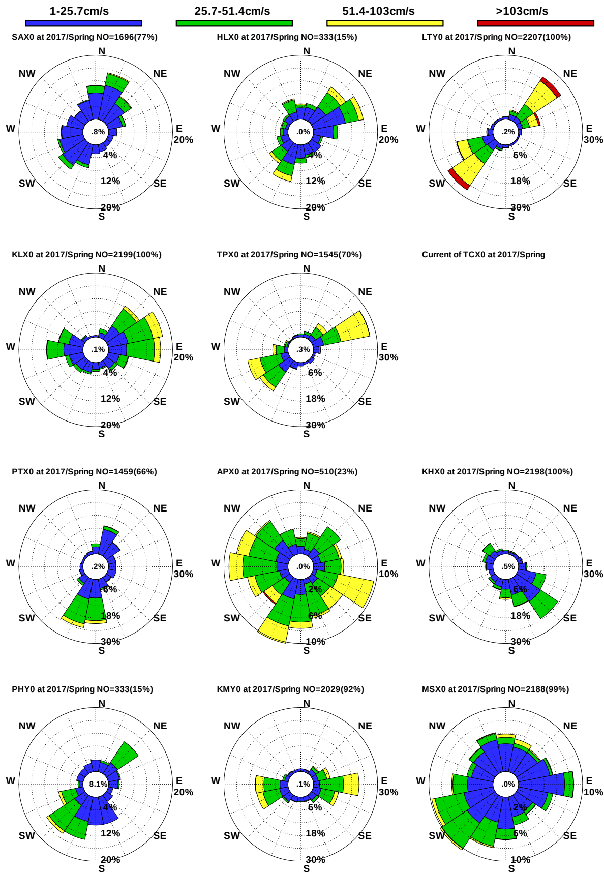
圖9.27 12港域2017年春季觀測海流玫瑰比較圖
