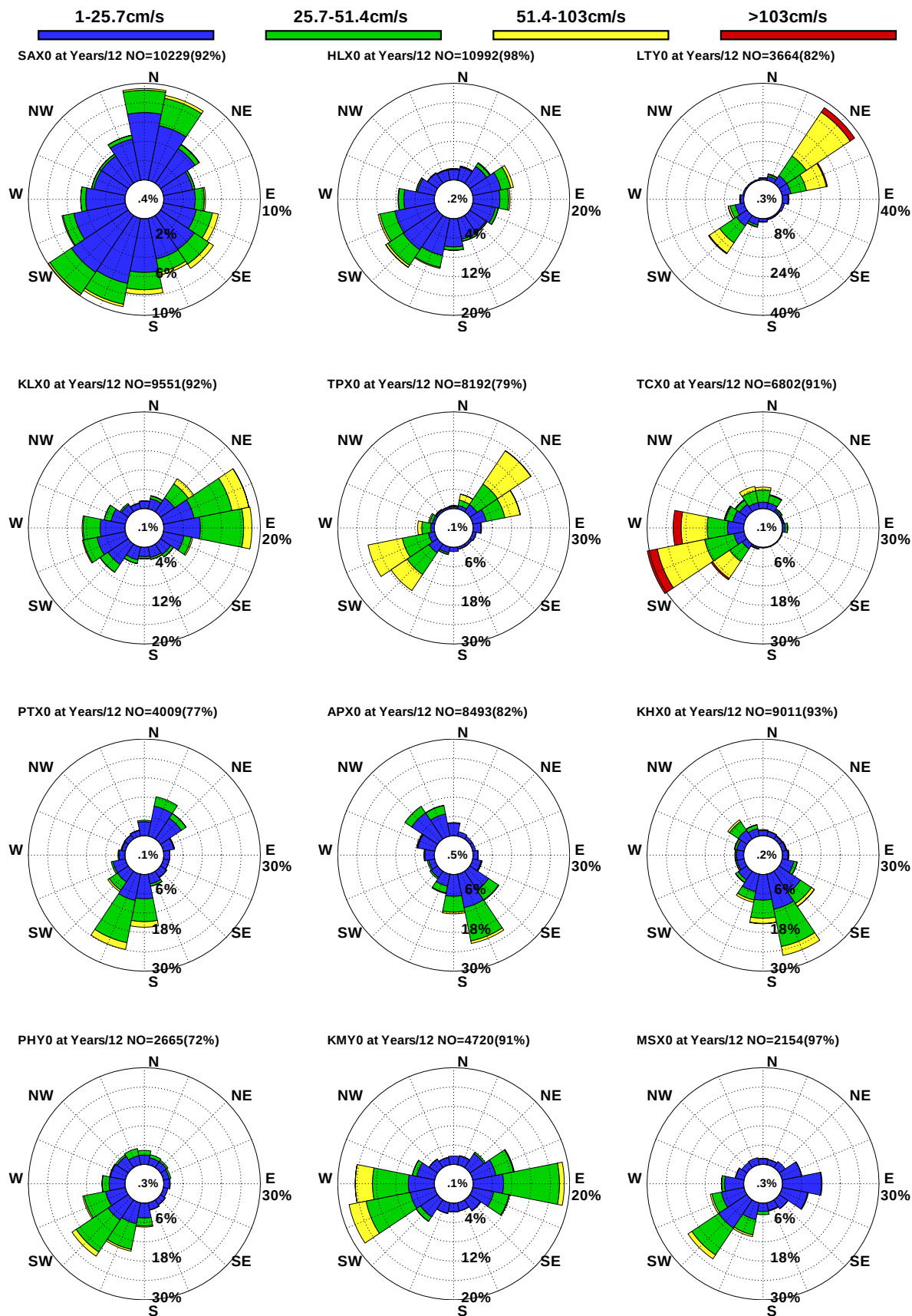
圖9.2 12港域歷年12月觀測海流玫瑰比較圖
