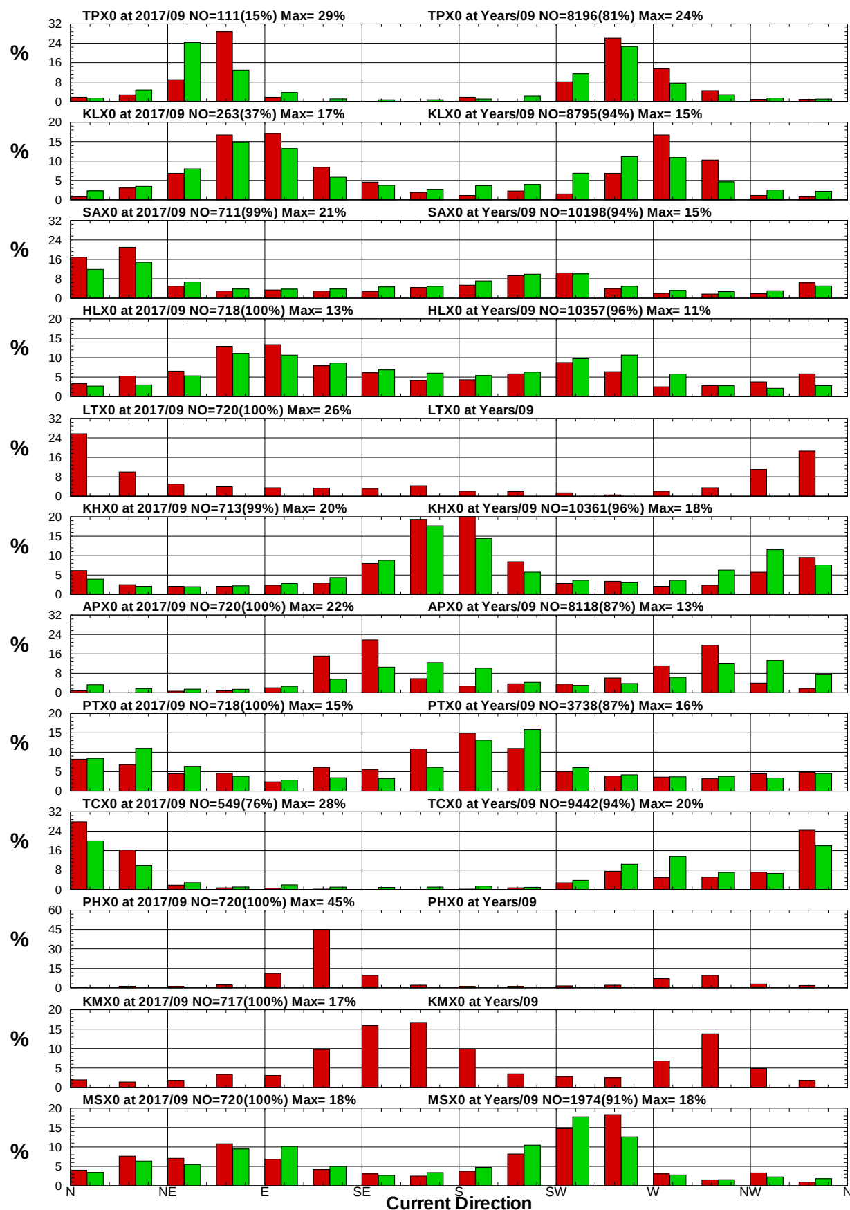
圖8.20 12港域2017年及歷年 9月流向統計方塊圖
