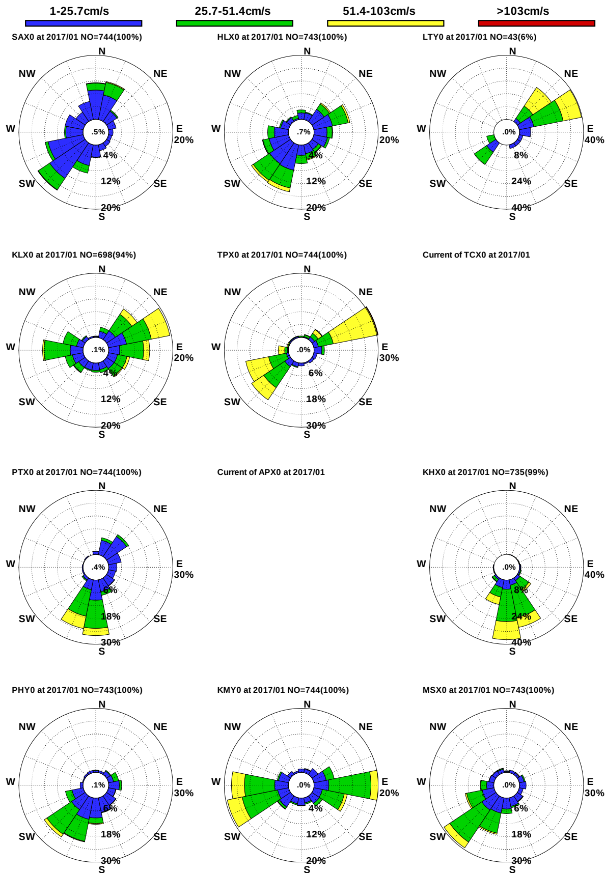
圖9.3 12港域2017年 1月觀測海流玫瑰比較圖
