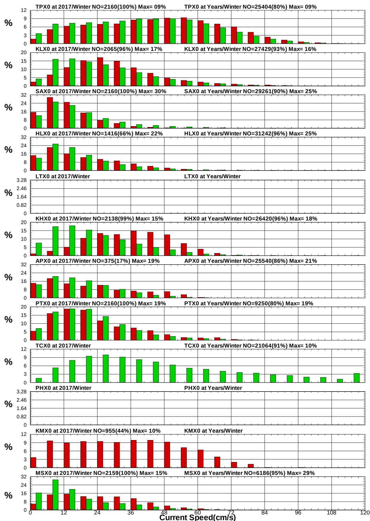
圖8.25 12港域2017年及歷年冬季流速統計方塊圖
