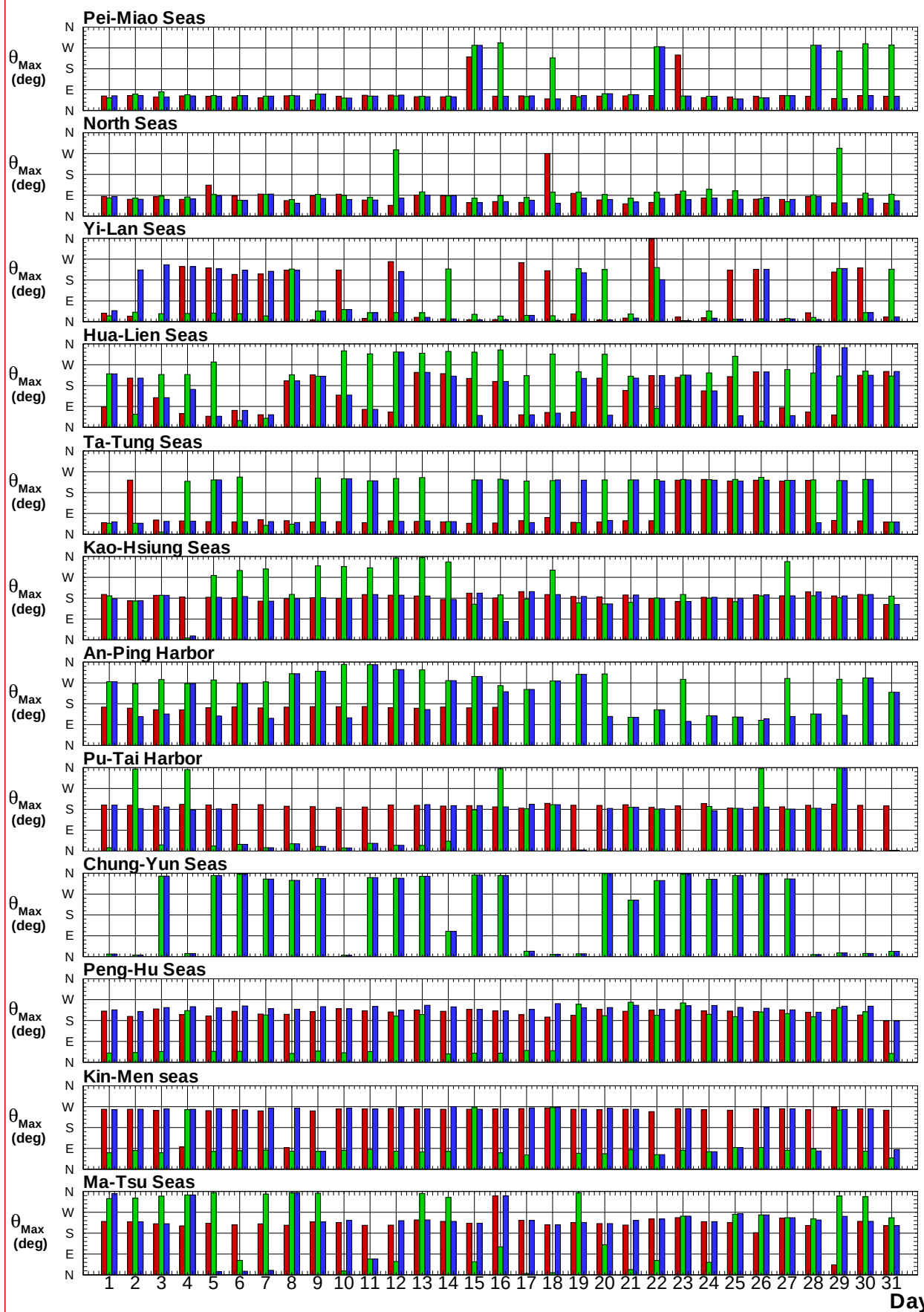
圖7.6d 2017年12港域冬, 夏及整年主要測站每日最大流速之流向圖
