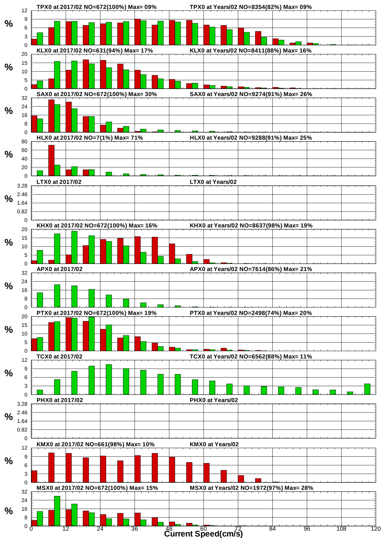
圖8.5 12港域2017年及歷年 2月流速統計方塊圖
