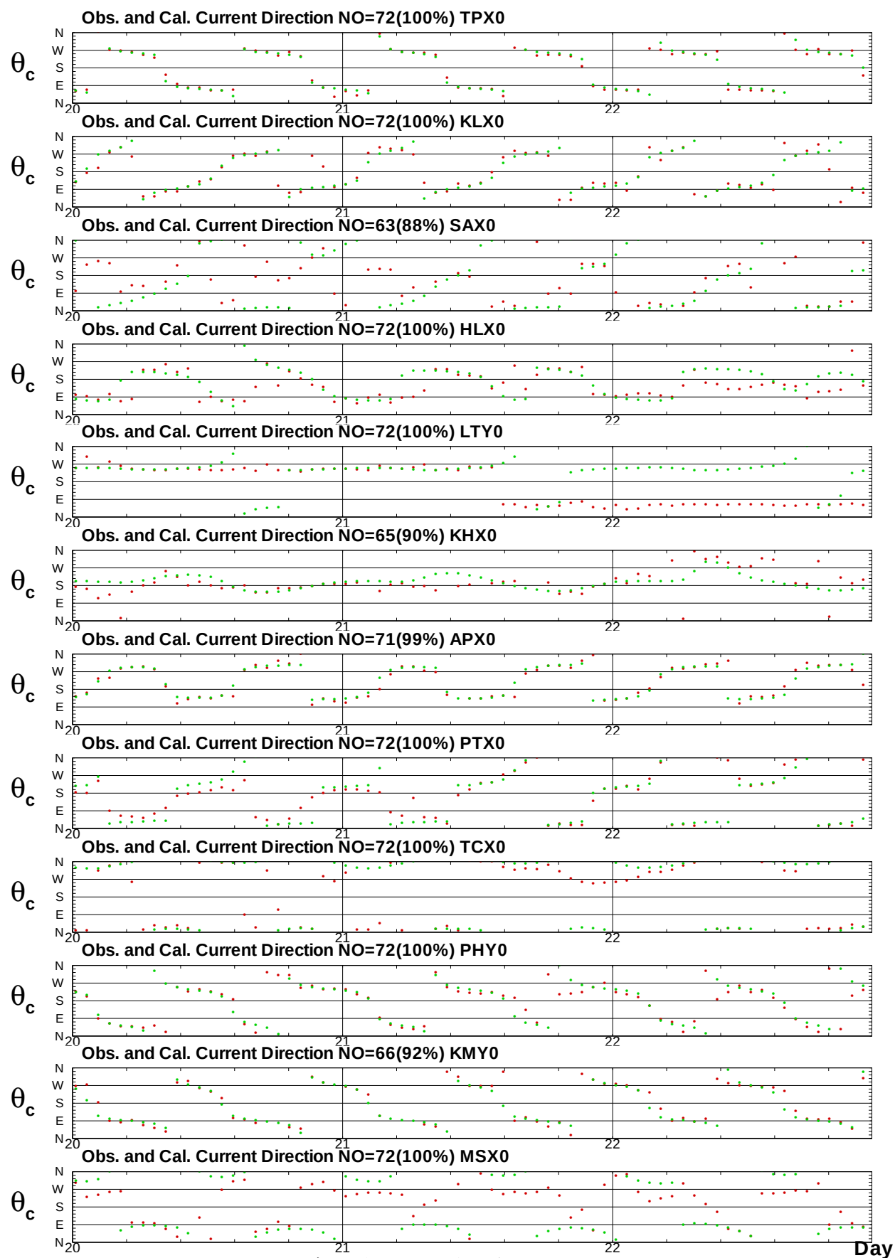
圖10.6 2017年天鵝 颱風12海域觀測流向歷線圖 (綠色: 潮流)
