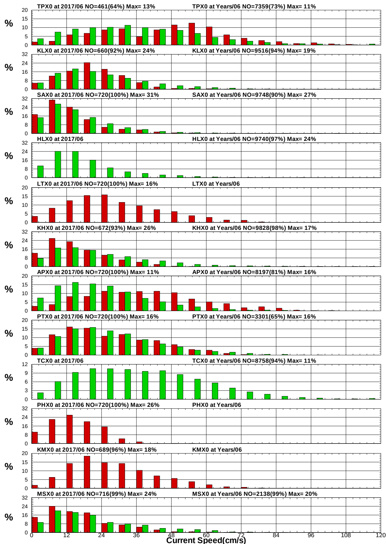
圖8.13 12港域2017年及歷年 6月流速統計方塊圖
