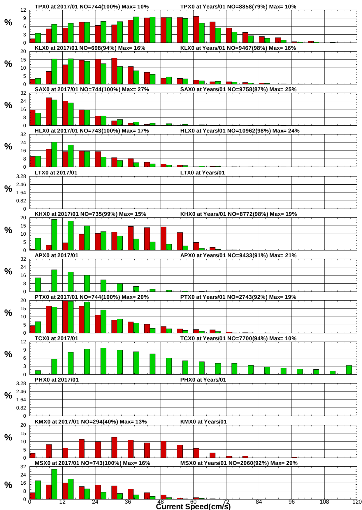
圖8.3 12港域2017年及歷年 1月流速統計方塊圖
