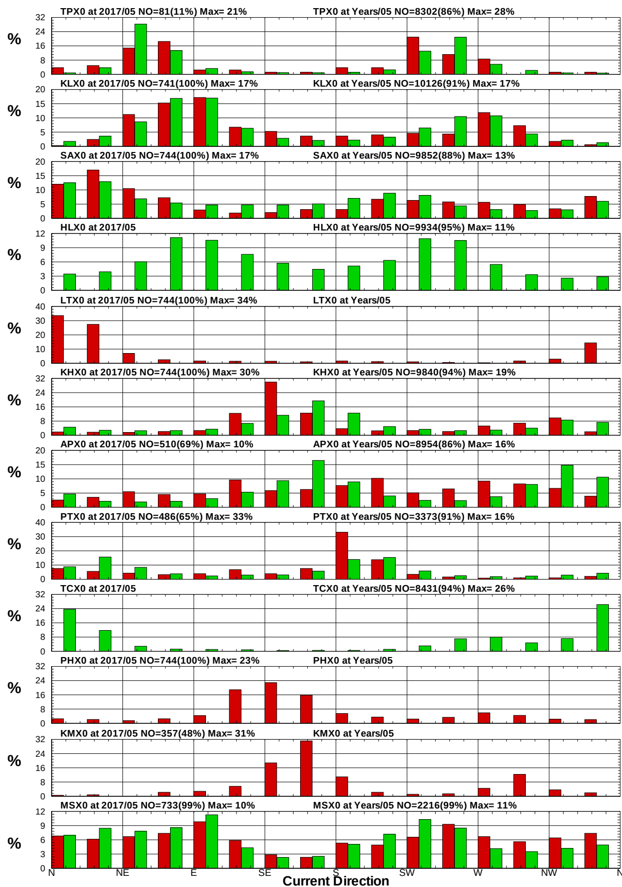
圖8.12 12港域2017年及歷年5月流向統計方塊圖
