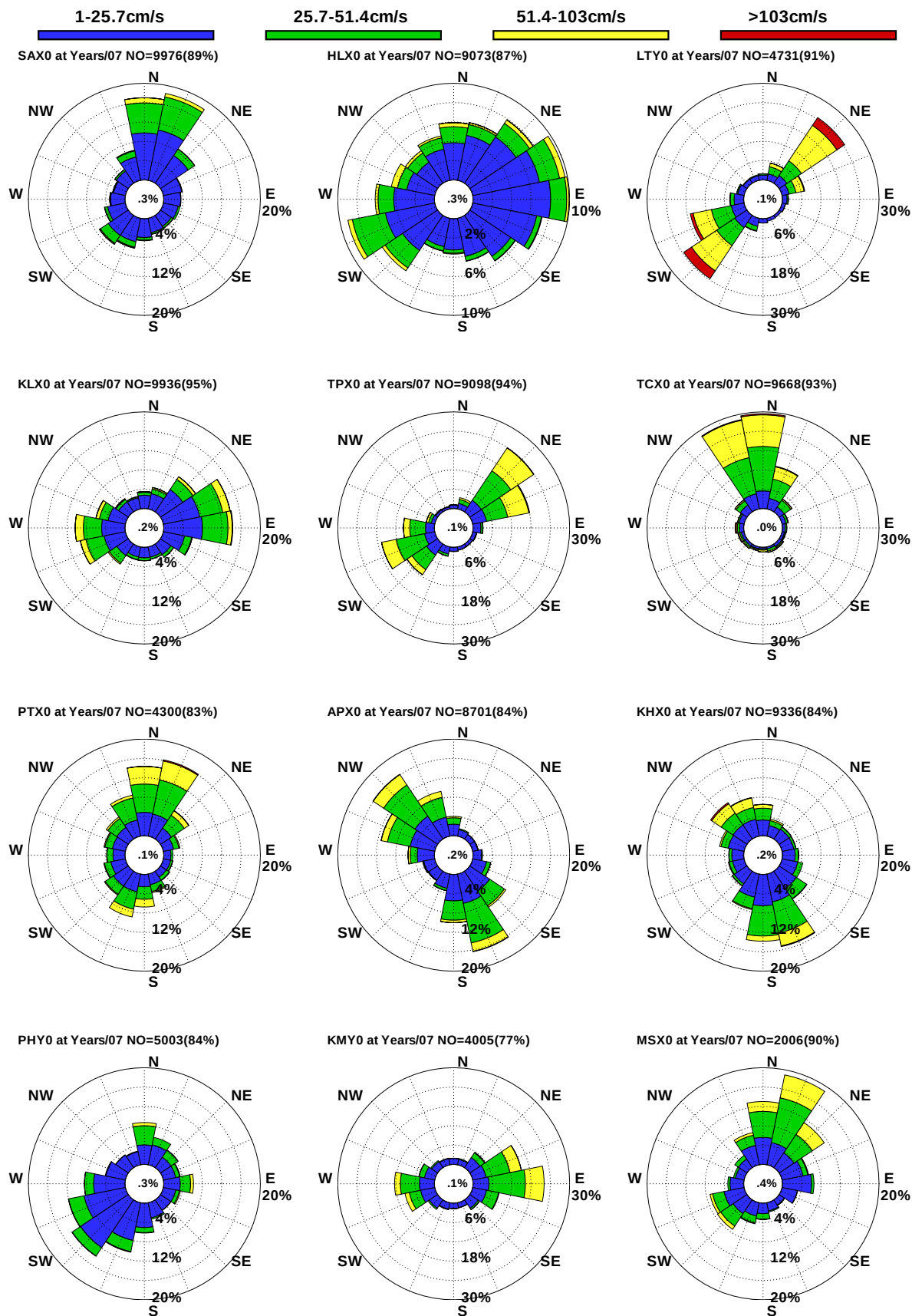
圖9.16 12港域歷年 7月觀測海流玫瑰比較圖
