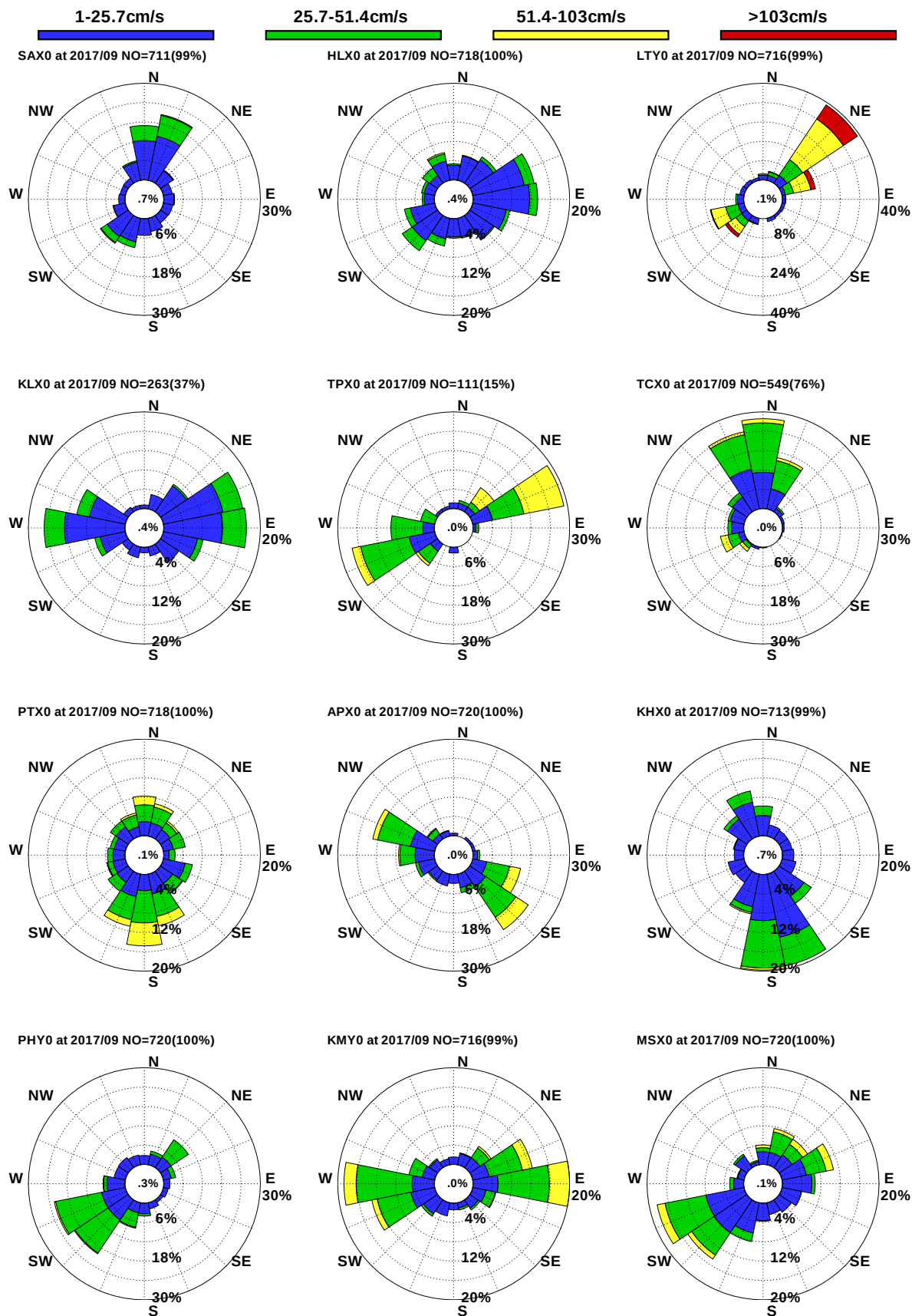
圖9.19 12港域2017年 9月觀測海流玫瑰比較圖
