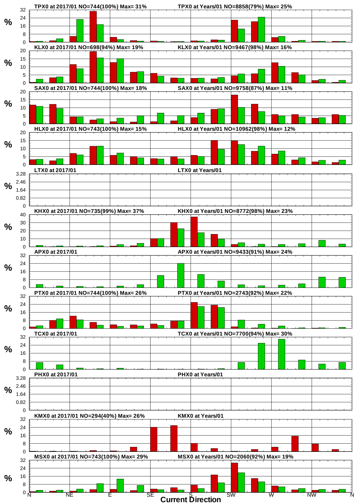
圖8.4 12港域2017年及歷年 1月流向統計方塊圖
