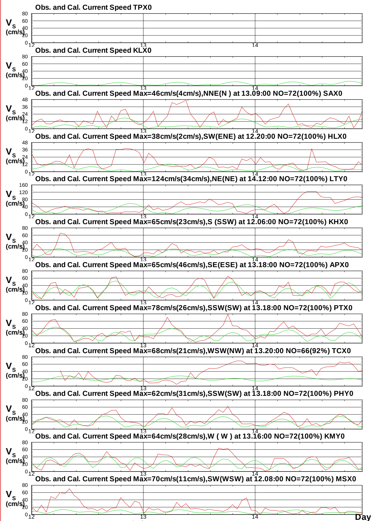
圖10.9 2017年泰利 颱風12海域觀測流速歷線圖 (綠色: 潮流)
