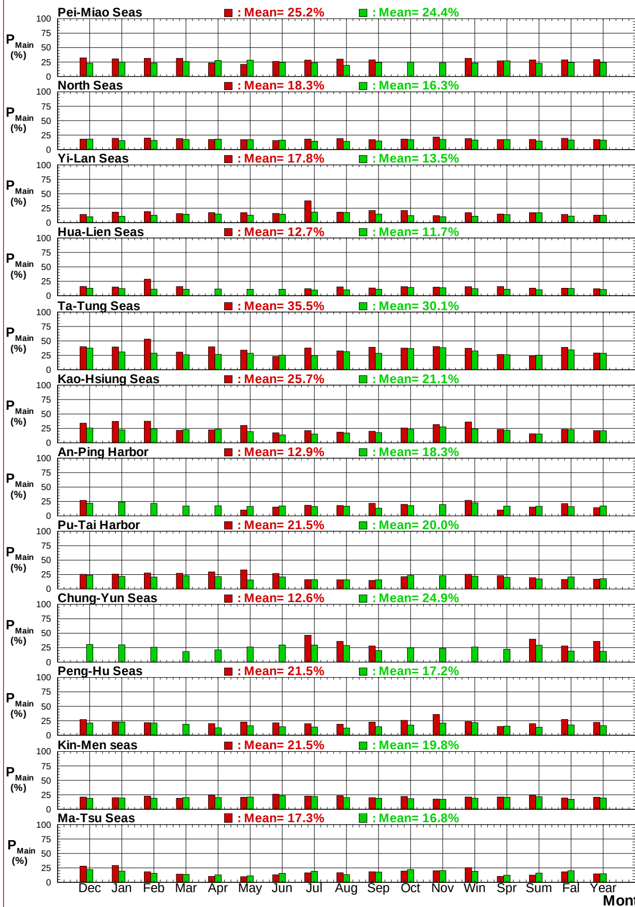
圖7.3f 2017及歷年12港域主要測站每月 (季) 主要流向百分比圖
