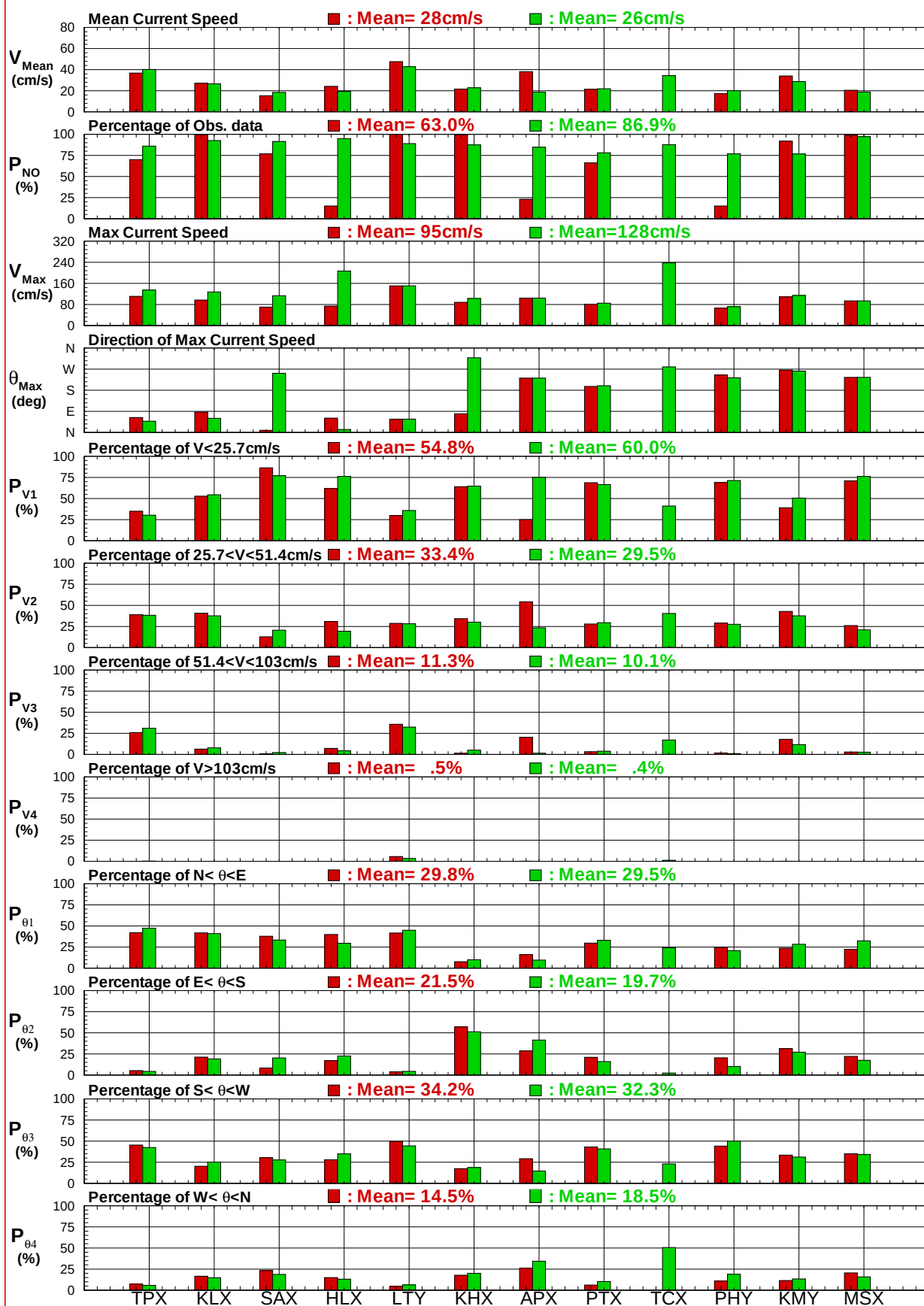
圖7.1b 12個港域2017及歷年主要測站春季流速 (向) 比較圖
