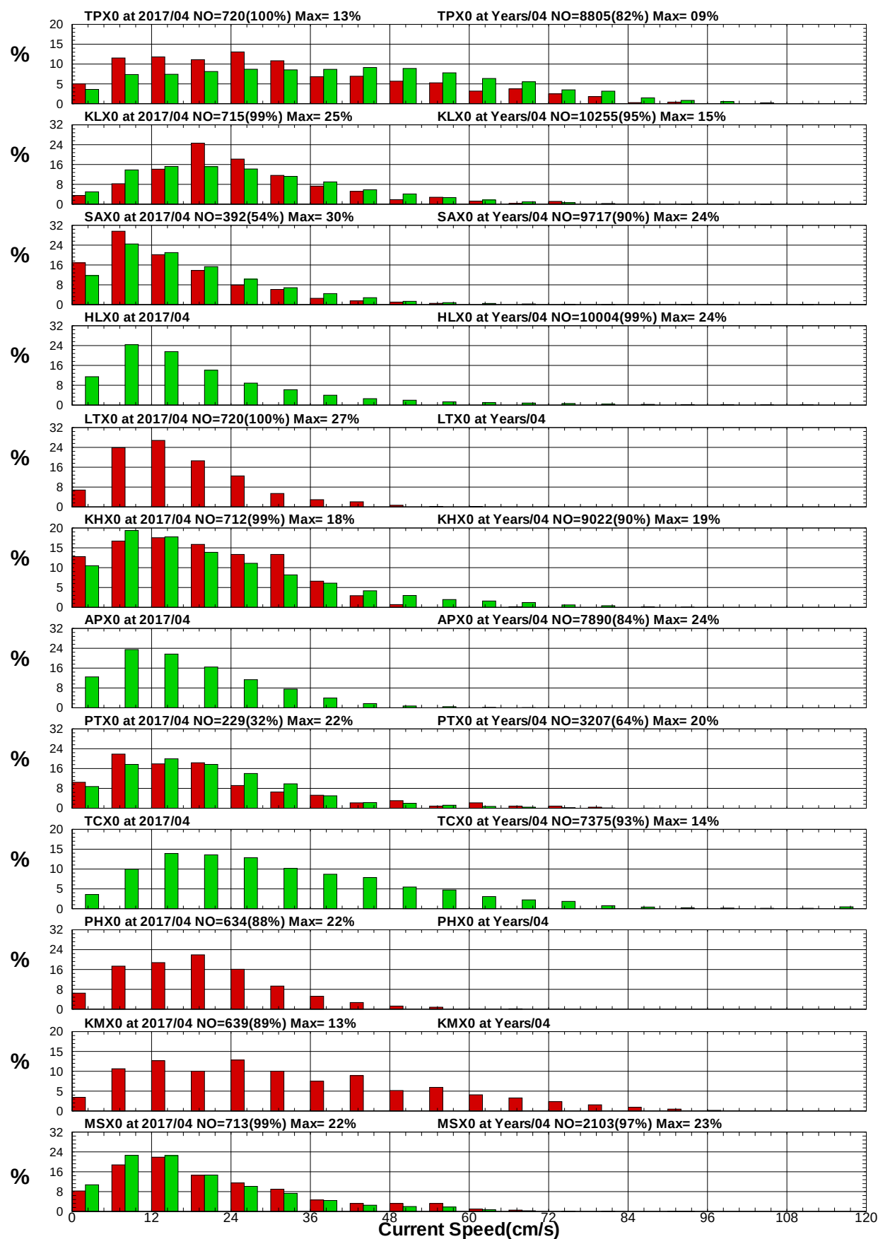
圖8.9 12港域2017年及歷年 4月流速統計方塊圖
