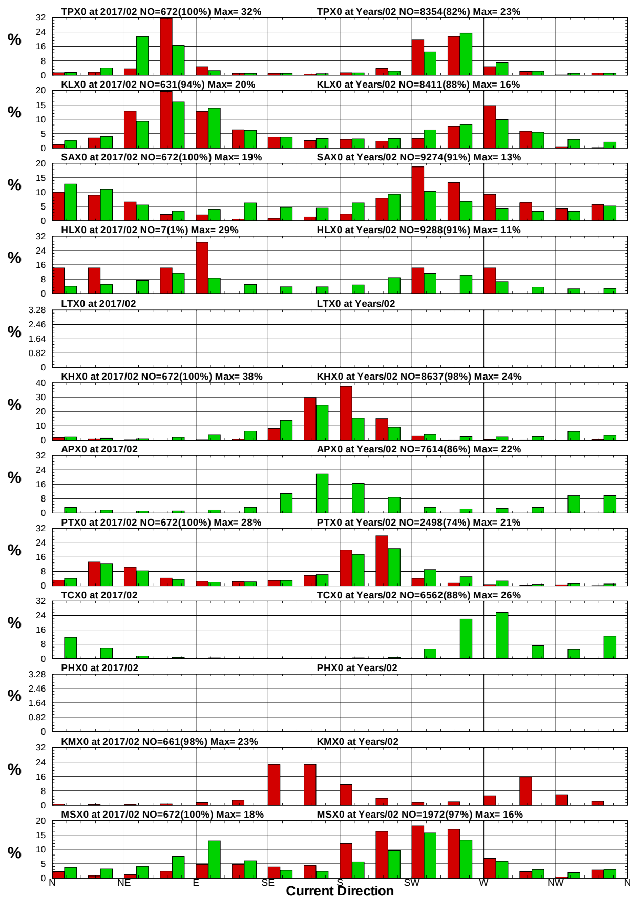
圖8.6 12港域2017年及歷年 2月流向統計方塊圖
