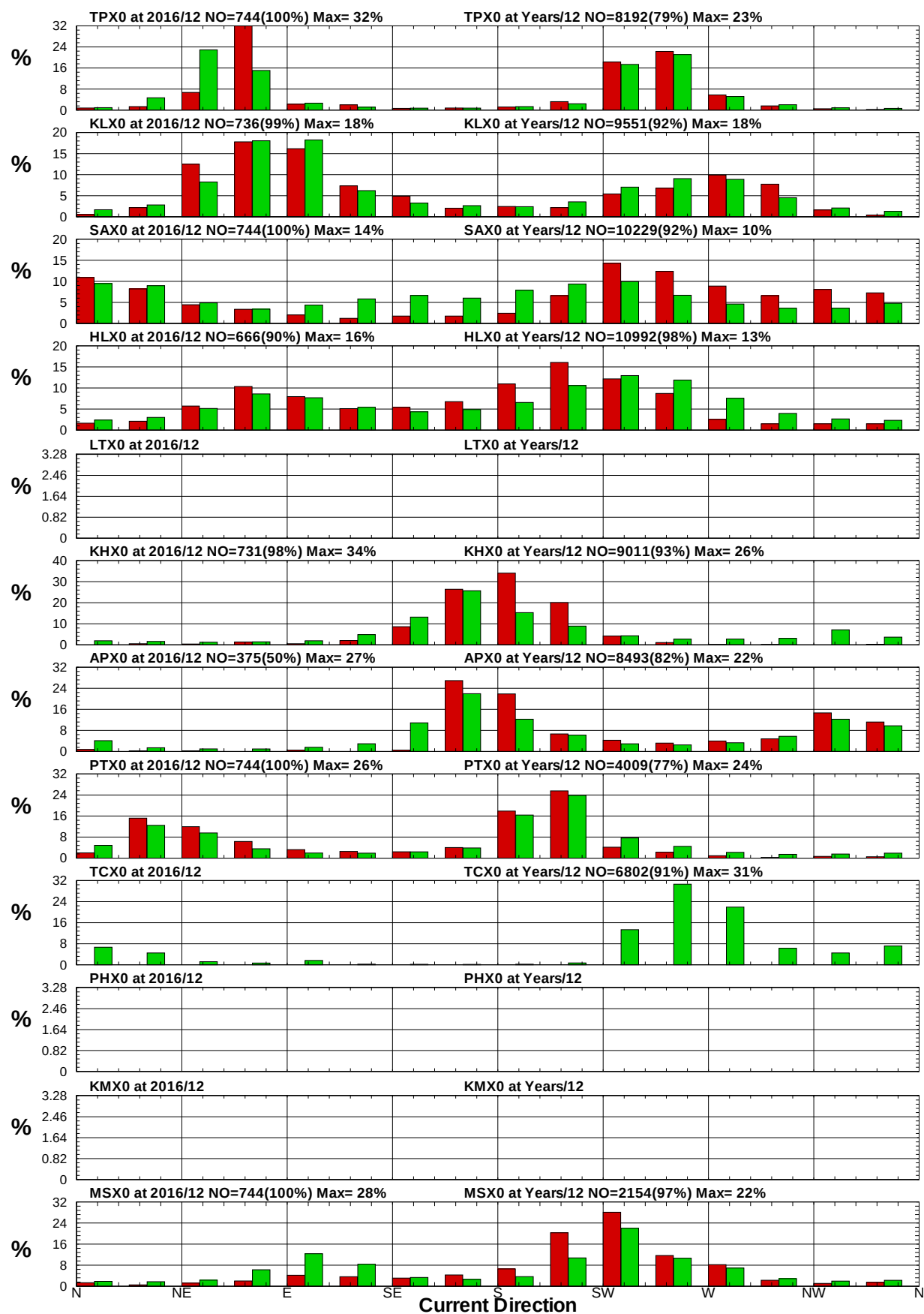
圖8.2 12港域2016年及歷年12月流向統計方塊圖
