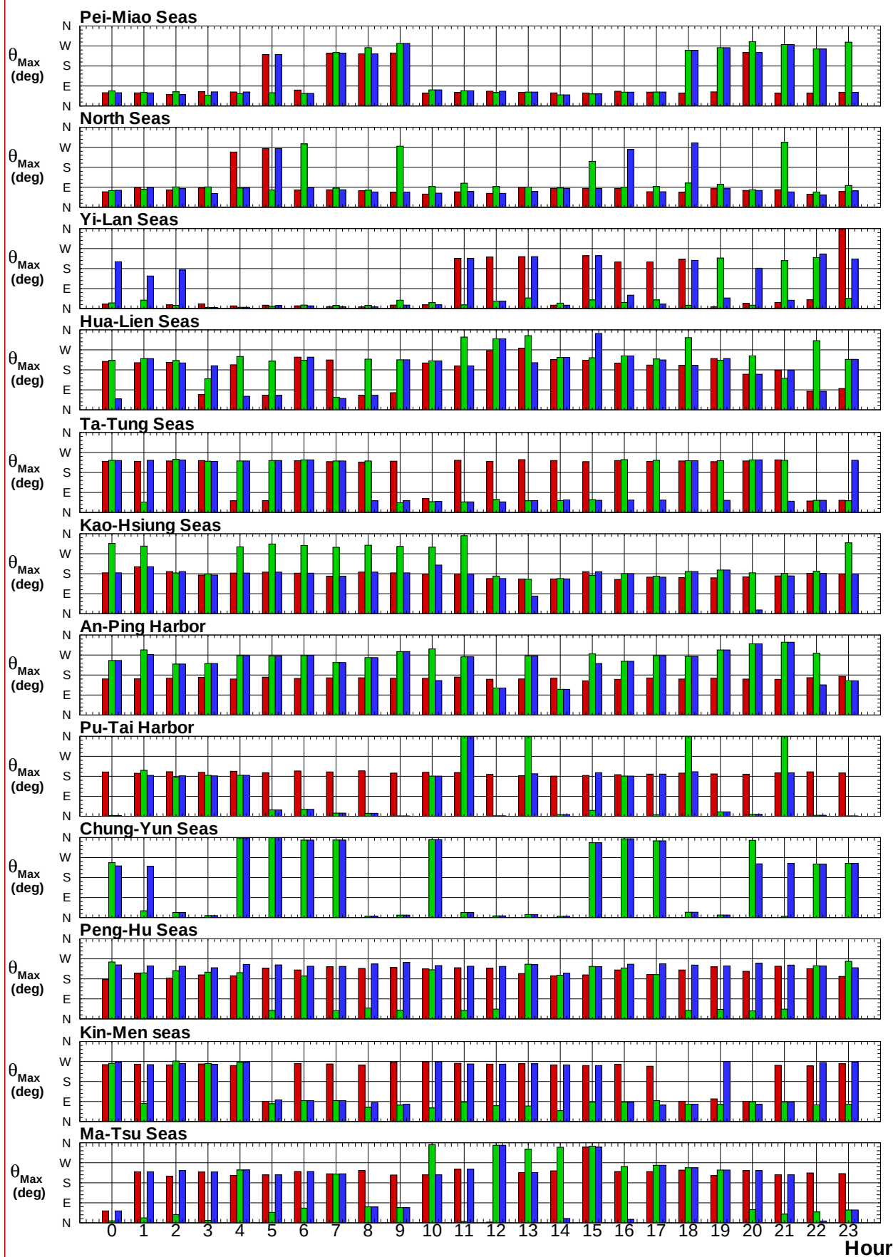
圖7.4d 2017年12港域冬, 夏及整年主要測站逐時最大流速之流向圖
