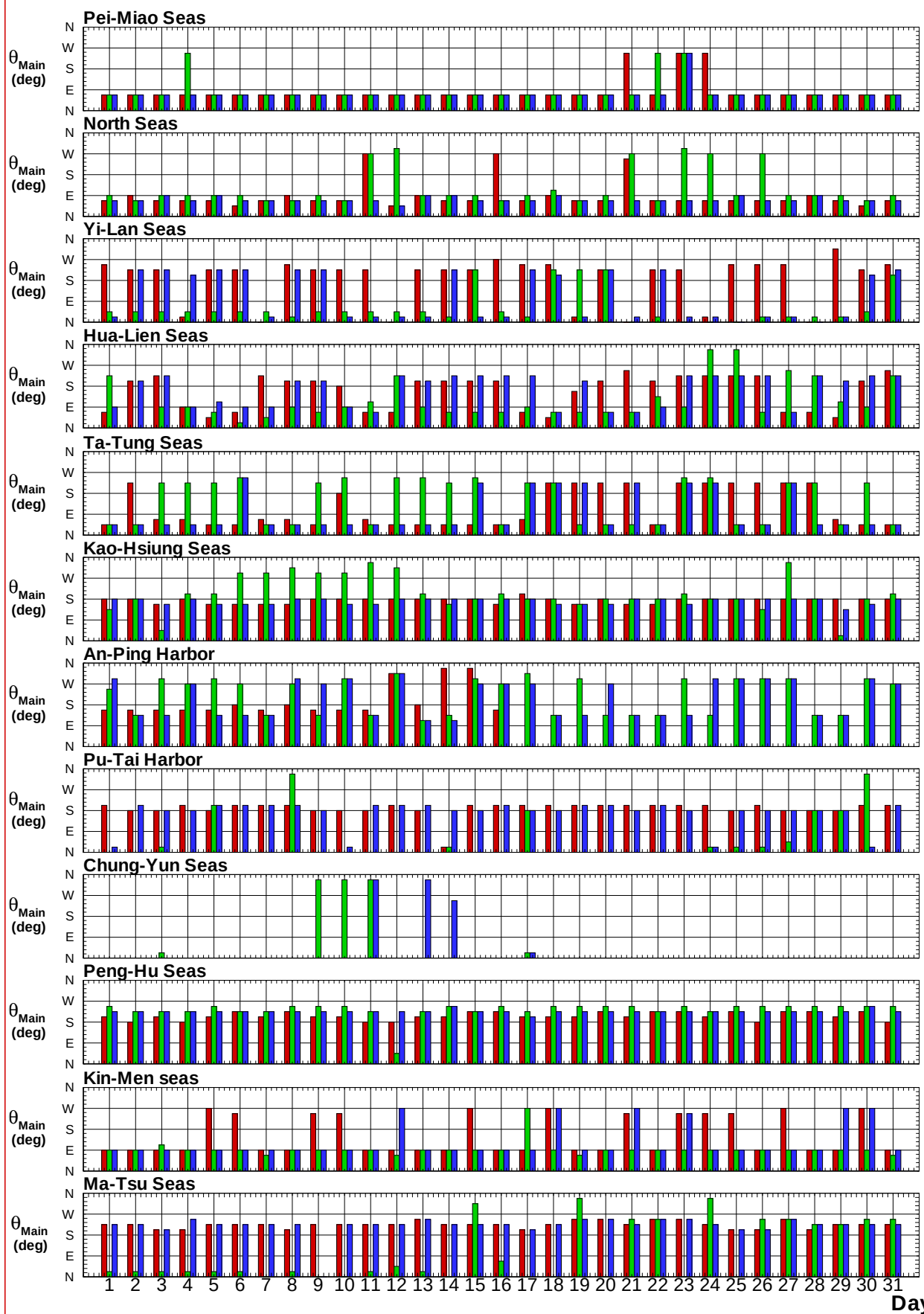
圖7.6e 2017年12港域冬, 夏及整年主要測站每日主要流向比較圖
