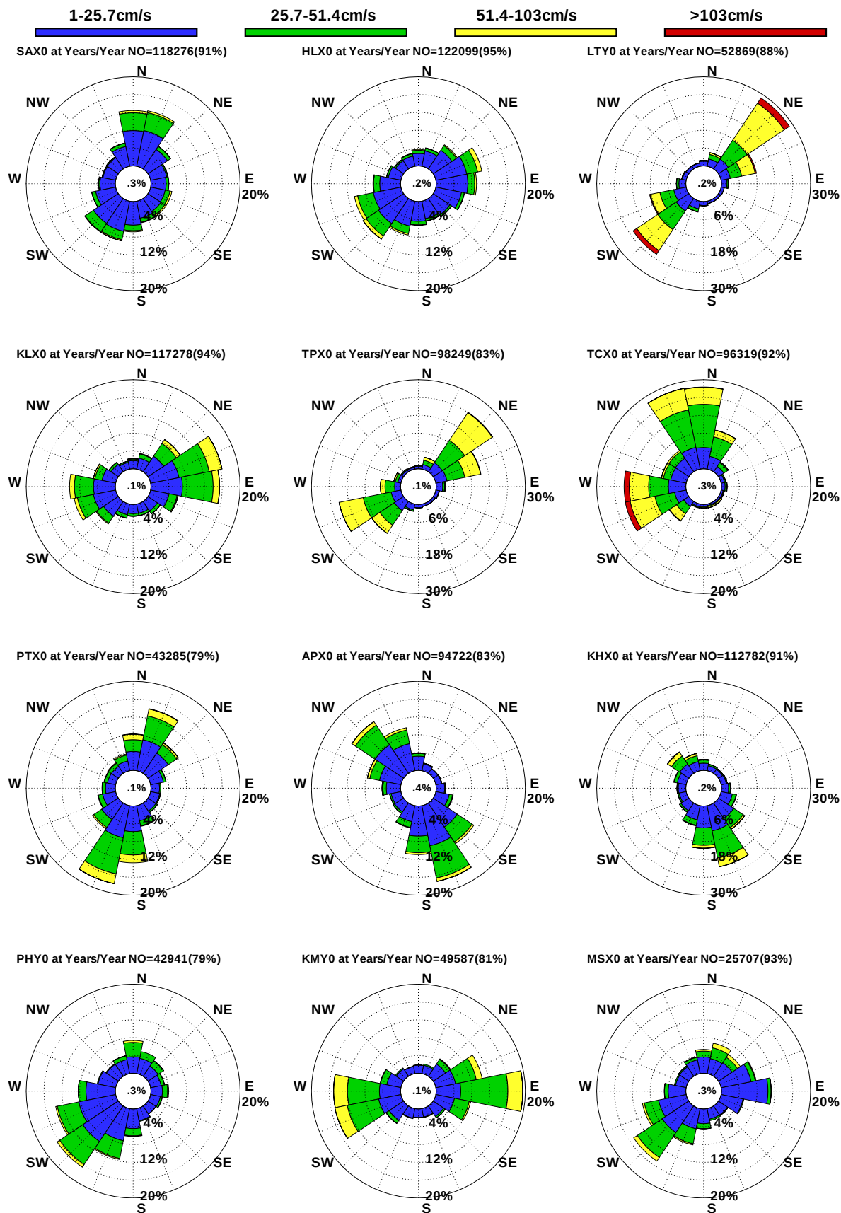
圖9.34 12港域歷年整年觀測海流玫瑰比較圖
