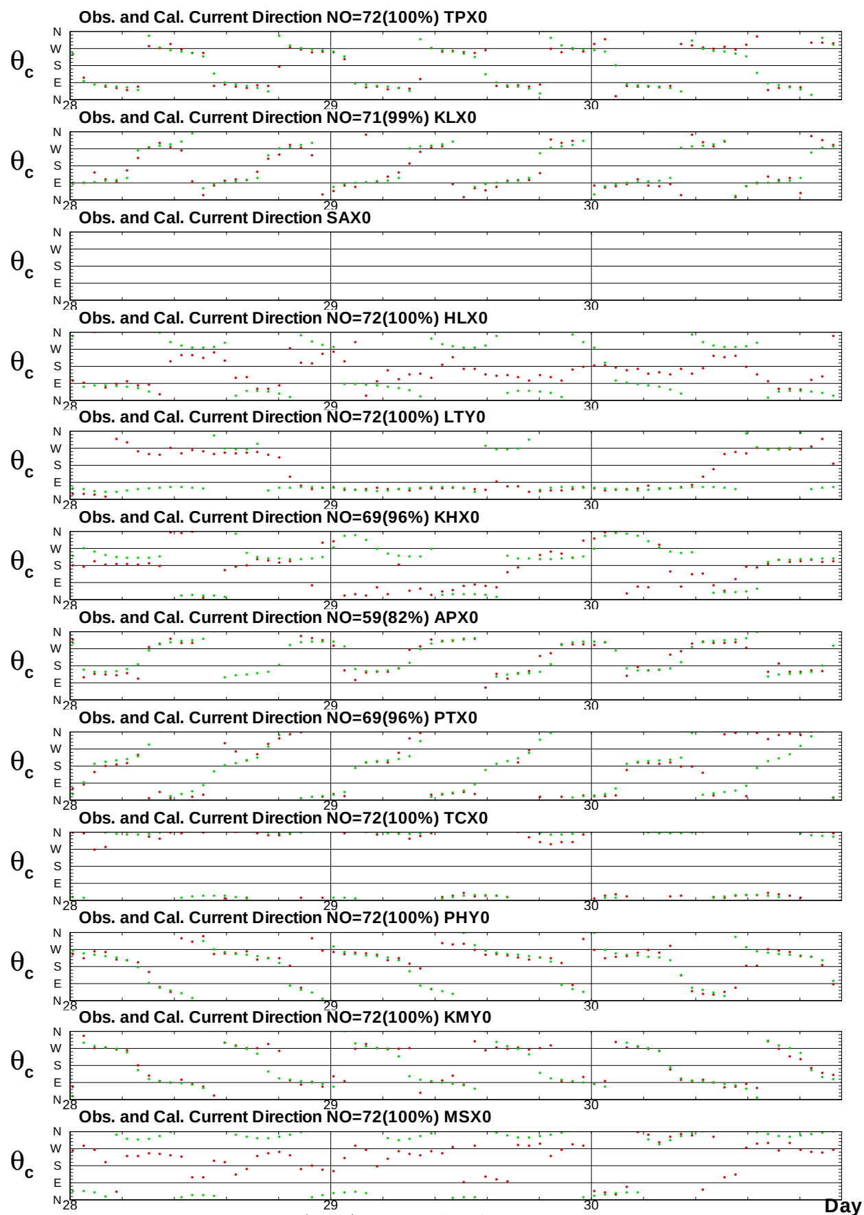
圖10.2 2017年尼莎 颱風12海域觀測流向歷線圖 (綠色: 潮流)
