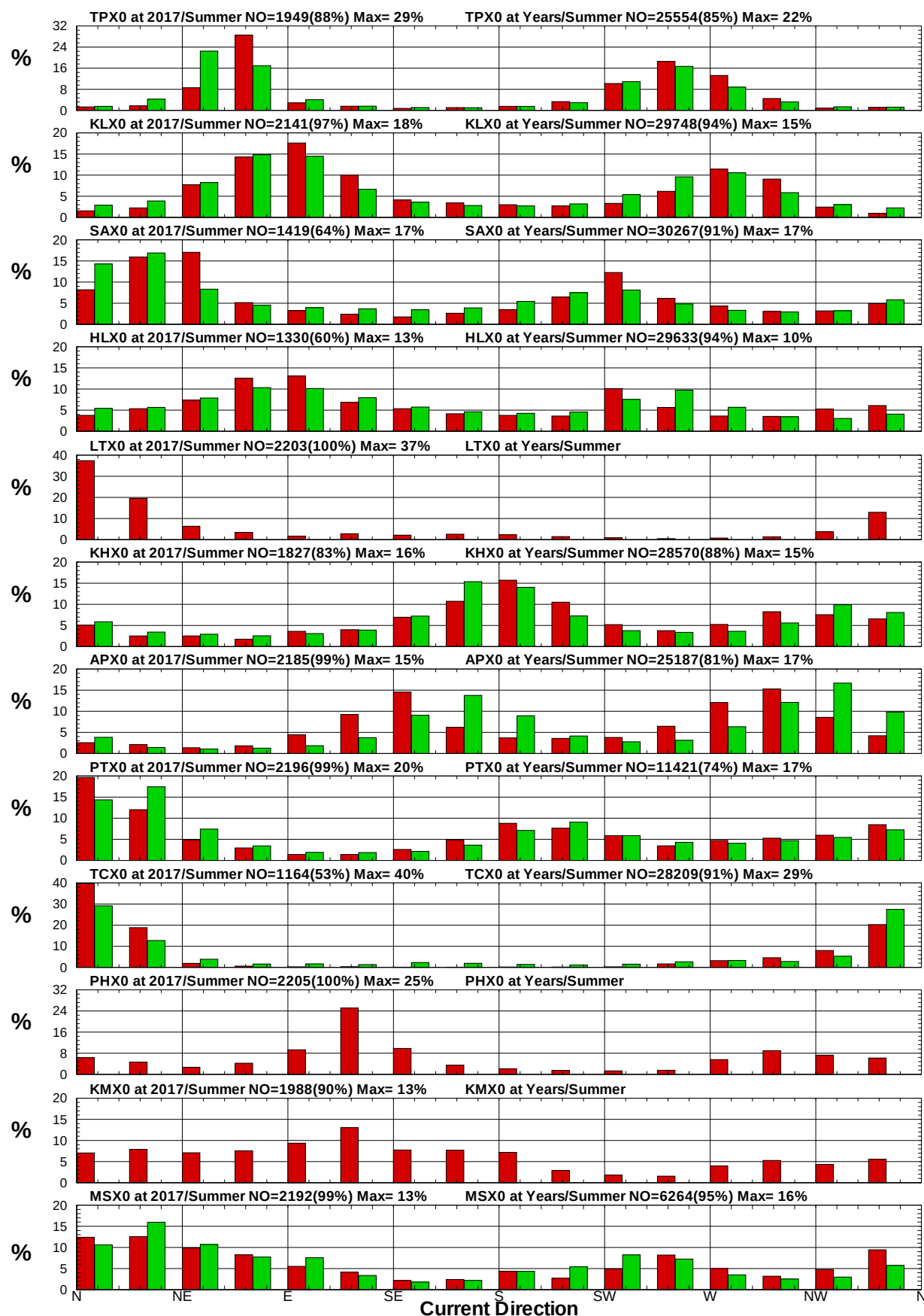
圖8.30 12港域2017年及歷年夏季流向統計方塊圖
