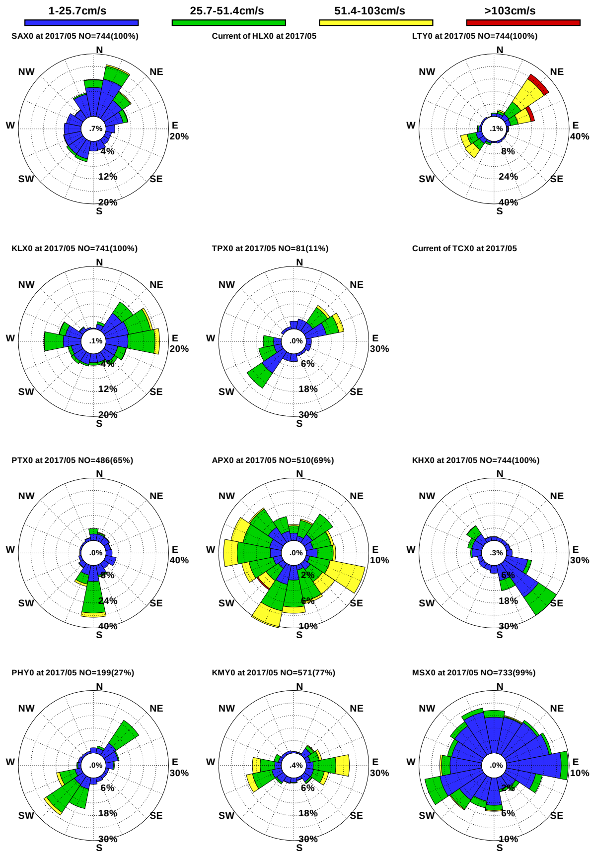
圖9.11 12港域2017年 5月觀測海流玫瑰比較圖
