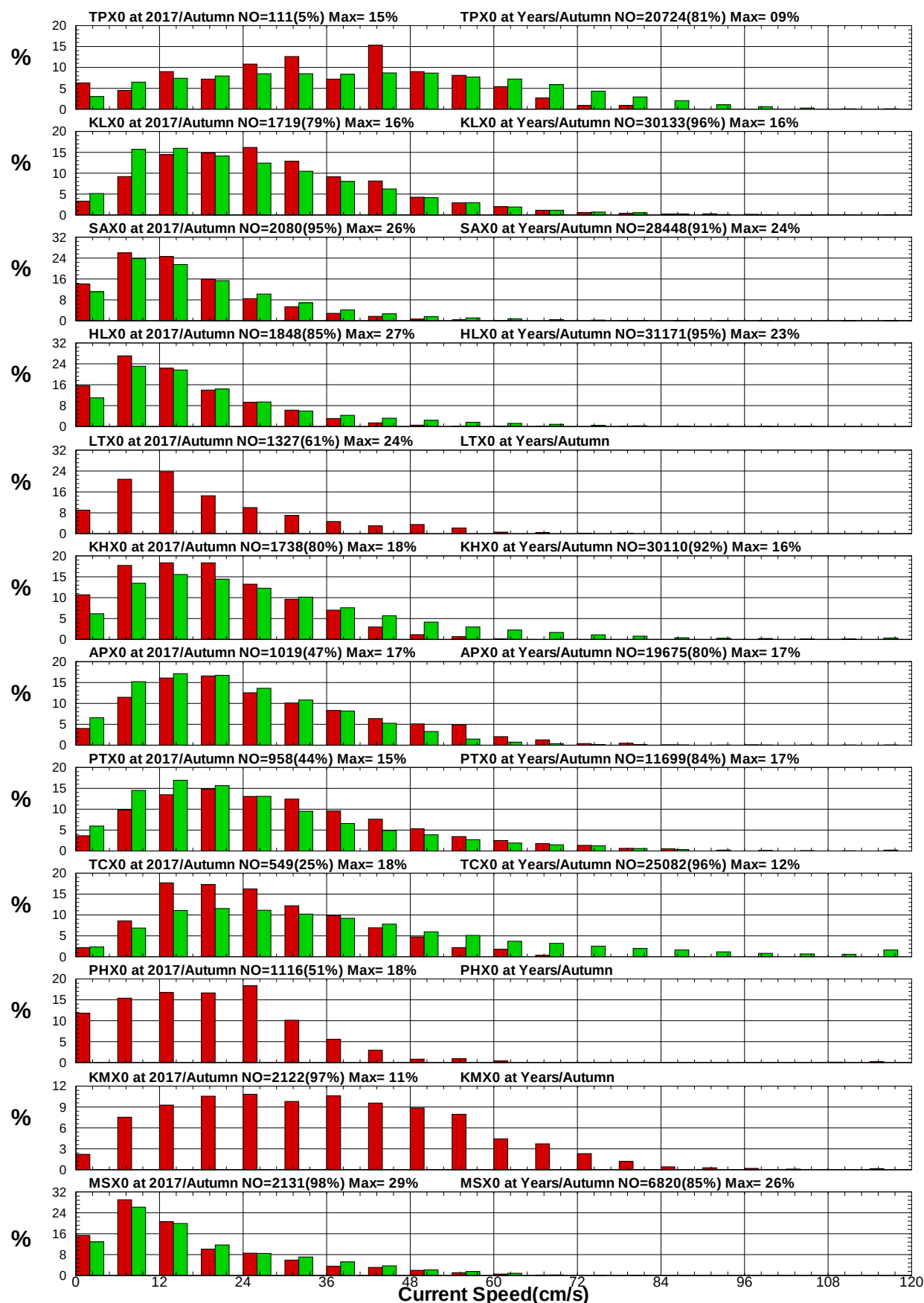
圖8.31 12港域2017年及歷年秋季流速統計方塊圖
