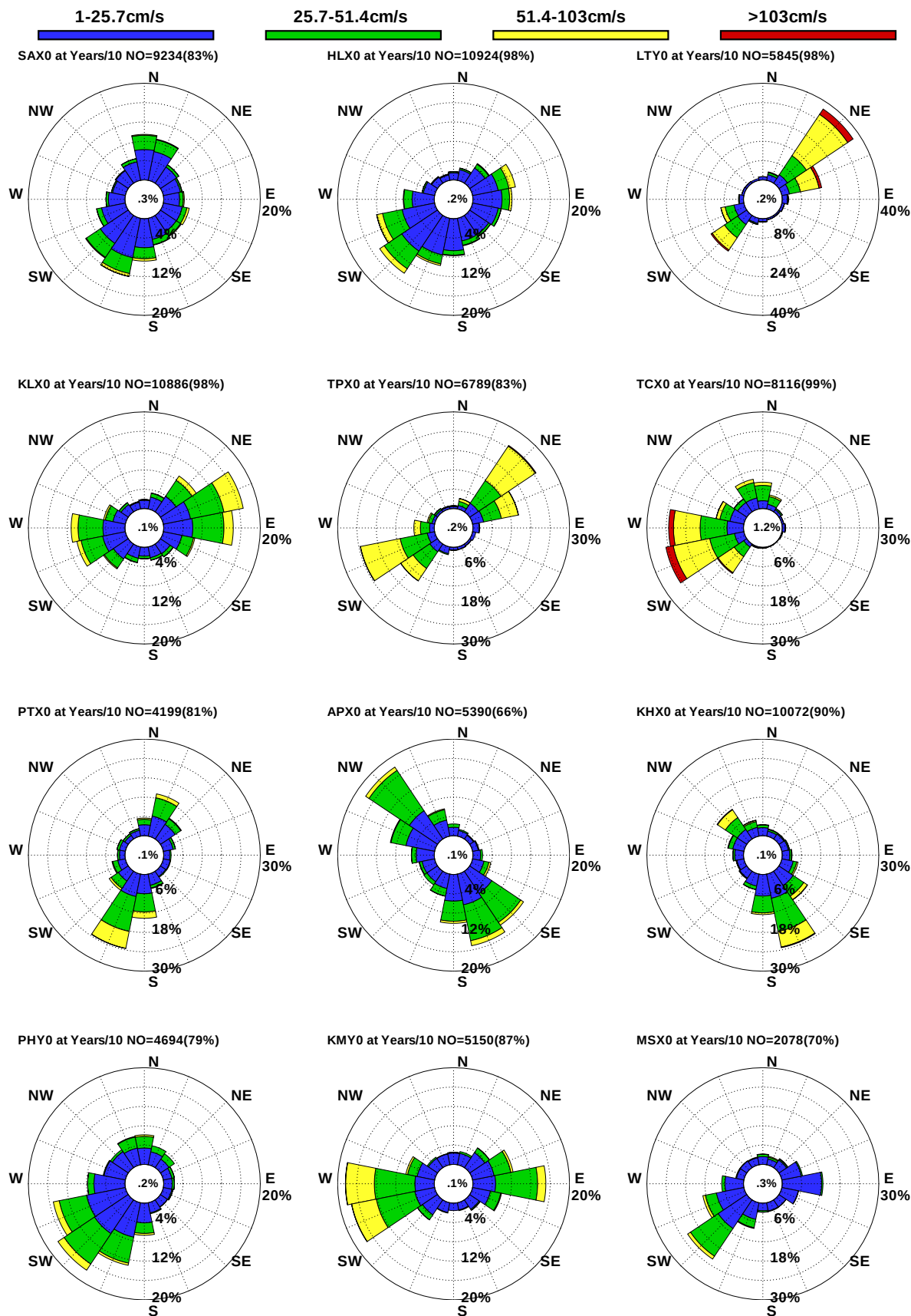
圖9.22 12港域歷年10月觀測海流玫瑰比較圖
