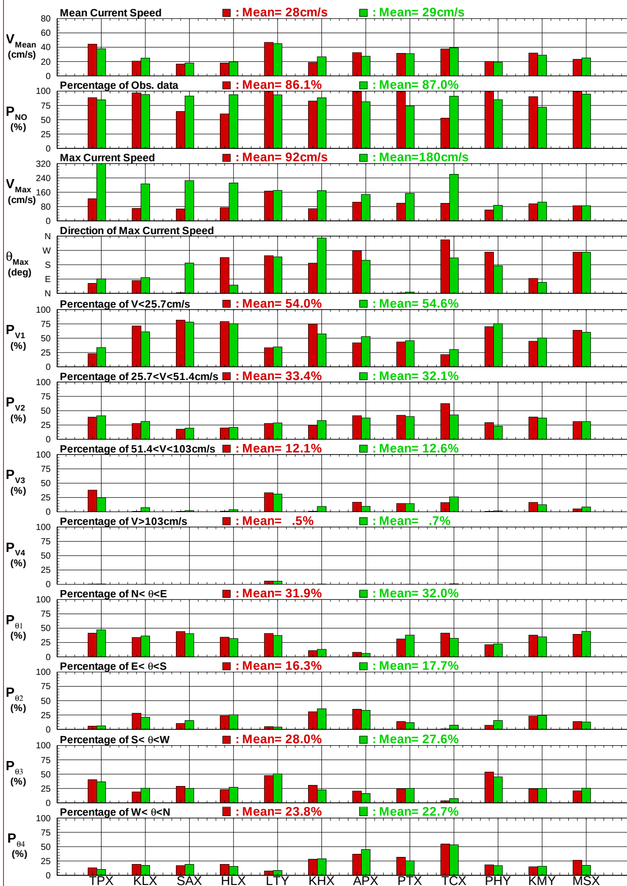
圖7.1c 12個港域2017及歷年主要測站夏季流速(向)比較圖
