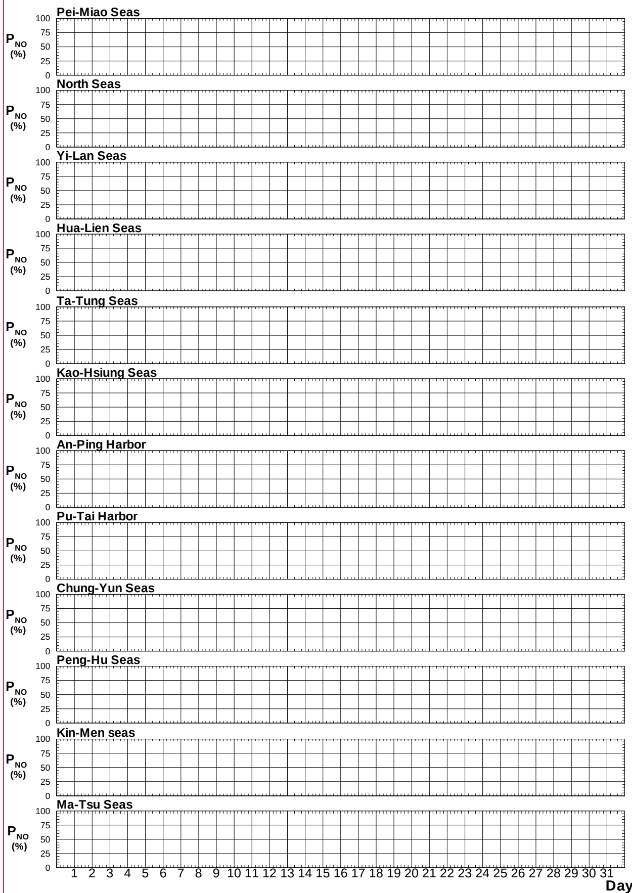
圖7.7b 歷年12港域冬, 夏及整年主要測站每日蒐集率比較圖
