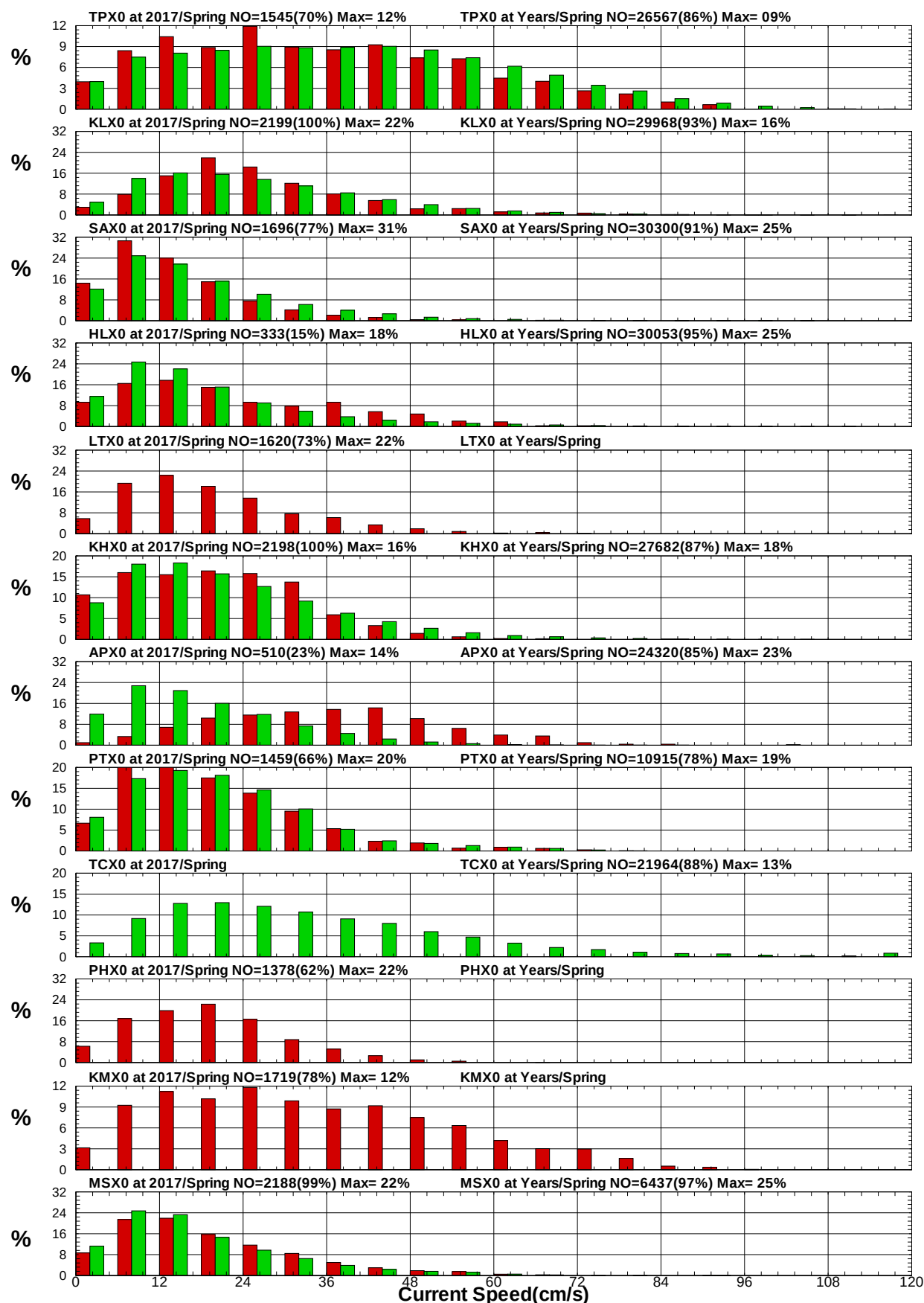
圖8.27 12港域2017年及歷年春季流速統計方塊圖
