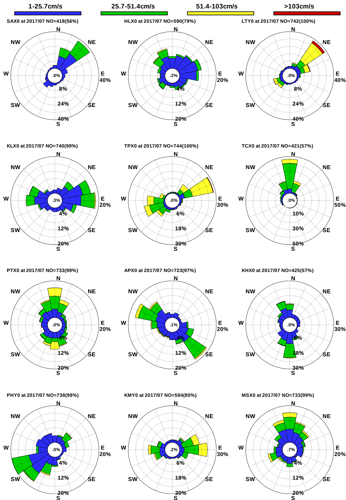
圖9.15 12港域2017年 7月觀測海流玫瑰比較圖
