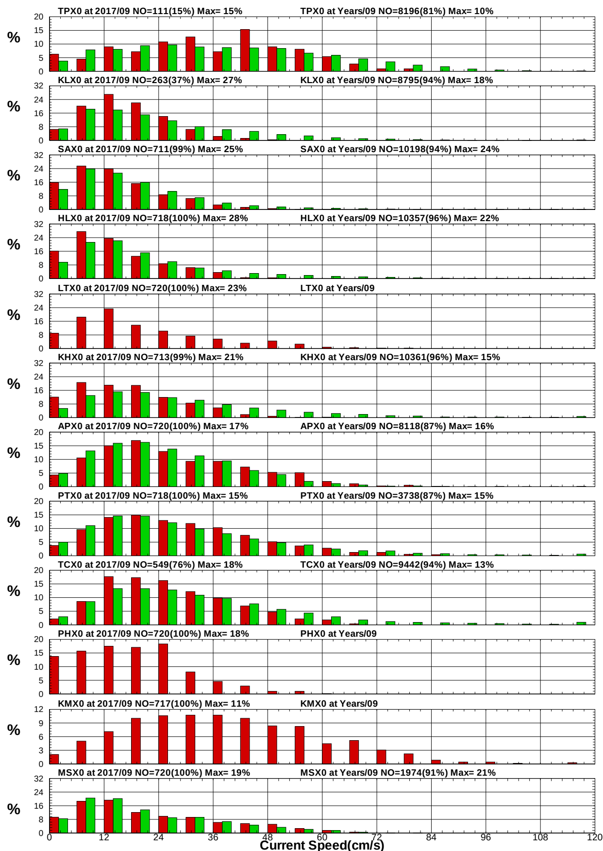
圖8.19 12港域2017年及歷年 9月流速統計方塊圖
