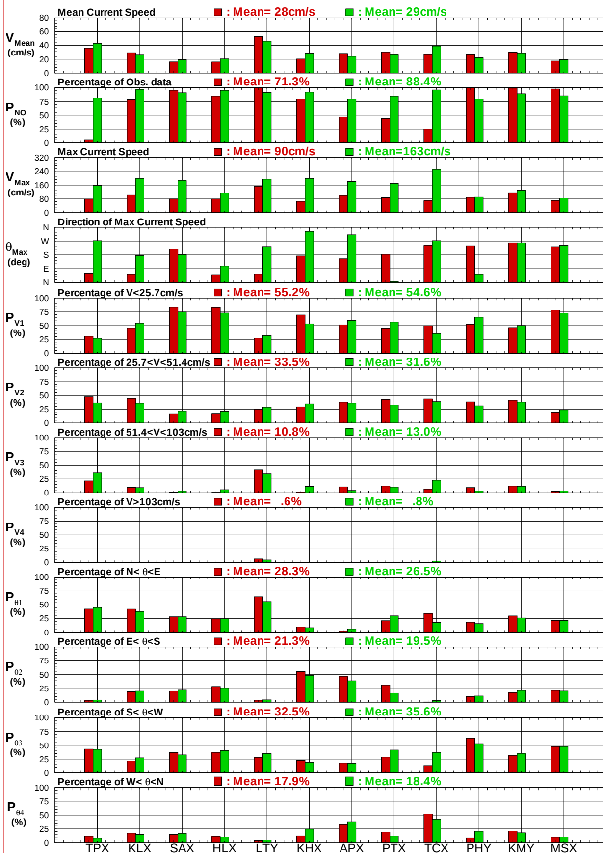
圖7.1d 12個港域2017及歷年主要測站秋季流速 (向) 比較圖
