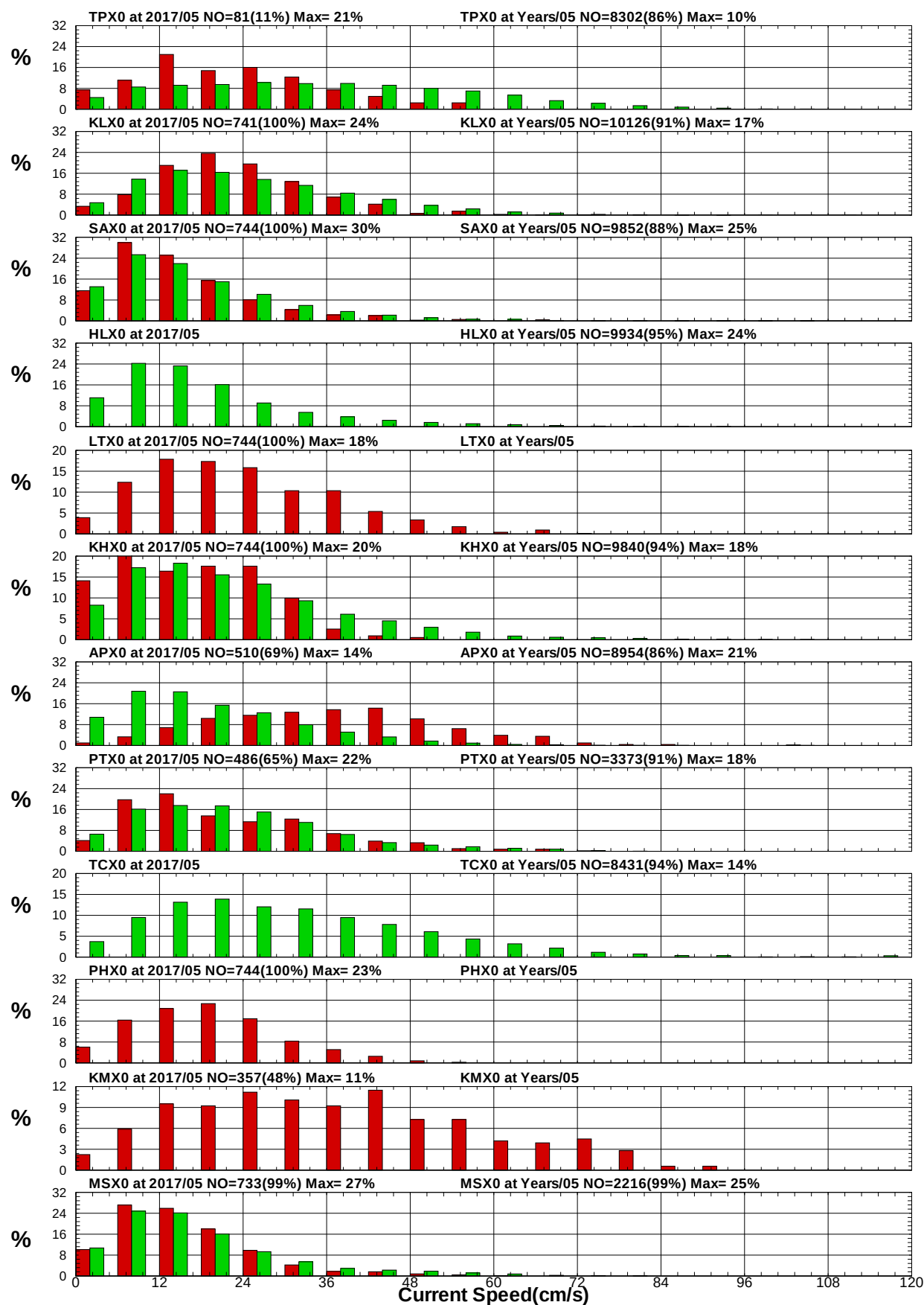
圖8.11 12港域2017年及歷年 5月流速統計方塊圖
