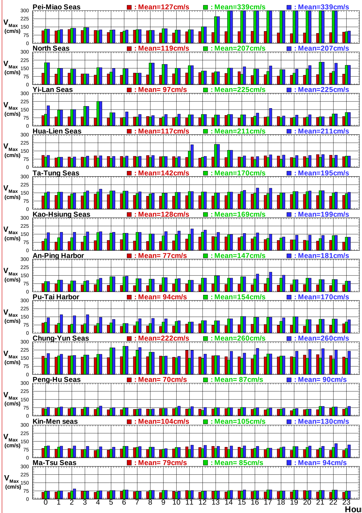
圖7.5c 歷年12港域冬, 夏及整年主要測站逐時最大流速比較圖
