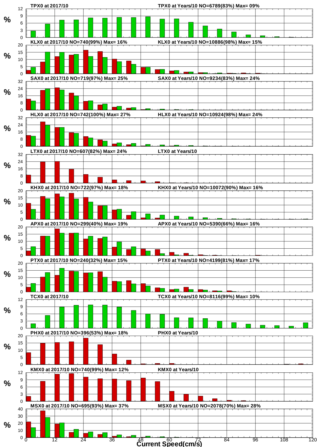
圖8.21 12港域2017年及歷年10月流速統計方塊圖
