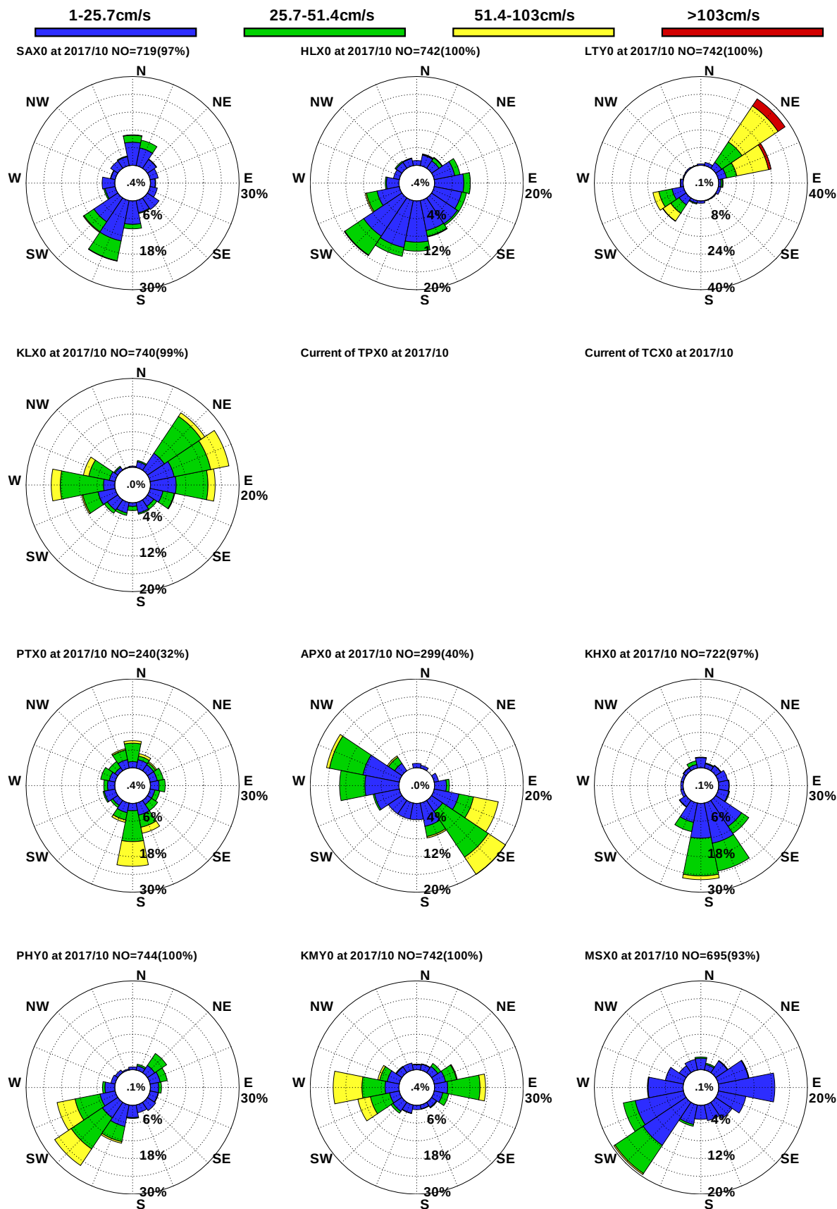
圖9.21 12港域2017年10月觀測海流玫瑰比較圖
