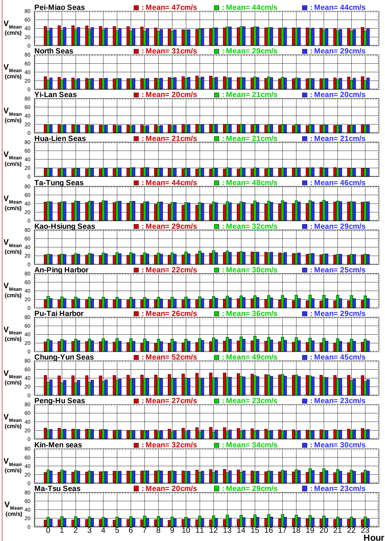
圖7.5a 歷年12港域冬, 夏及整年主要測站逐時平均流速比較圖
