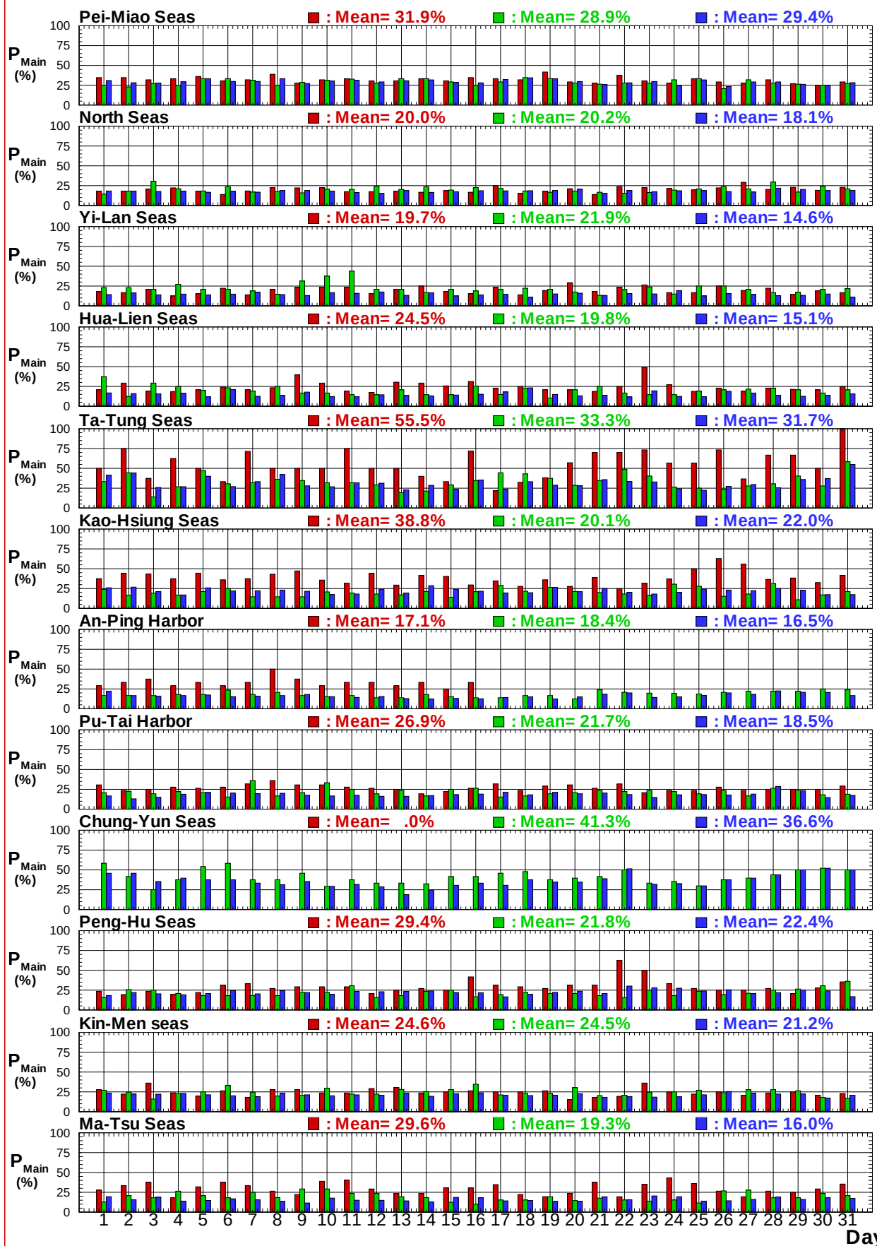
圖7.6f 2017年12港域冬, 夏及整年主要測站每日主要流向百分比圖
