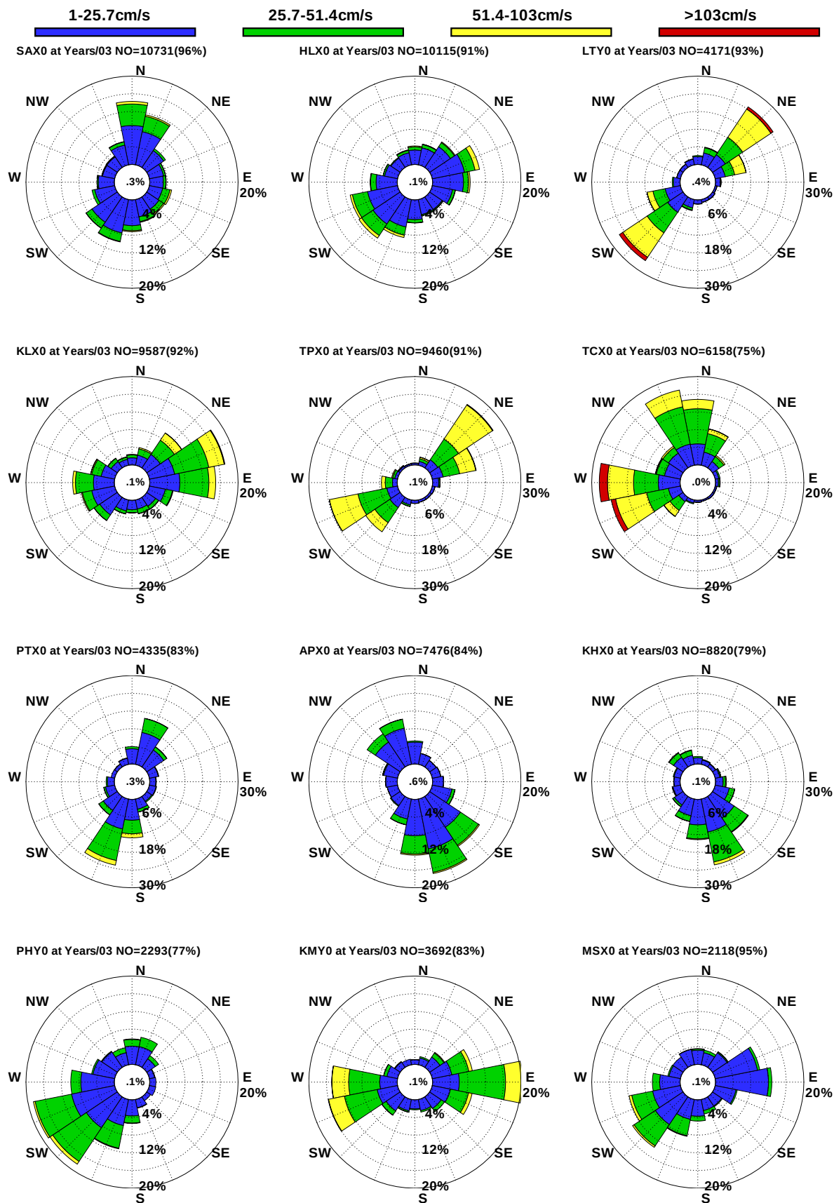
圖9.8 12港域歷年 3 月觀測海流玫瑰比較圖
