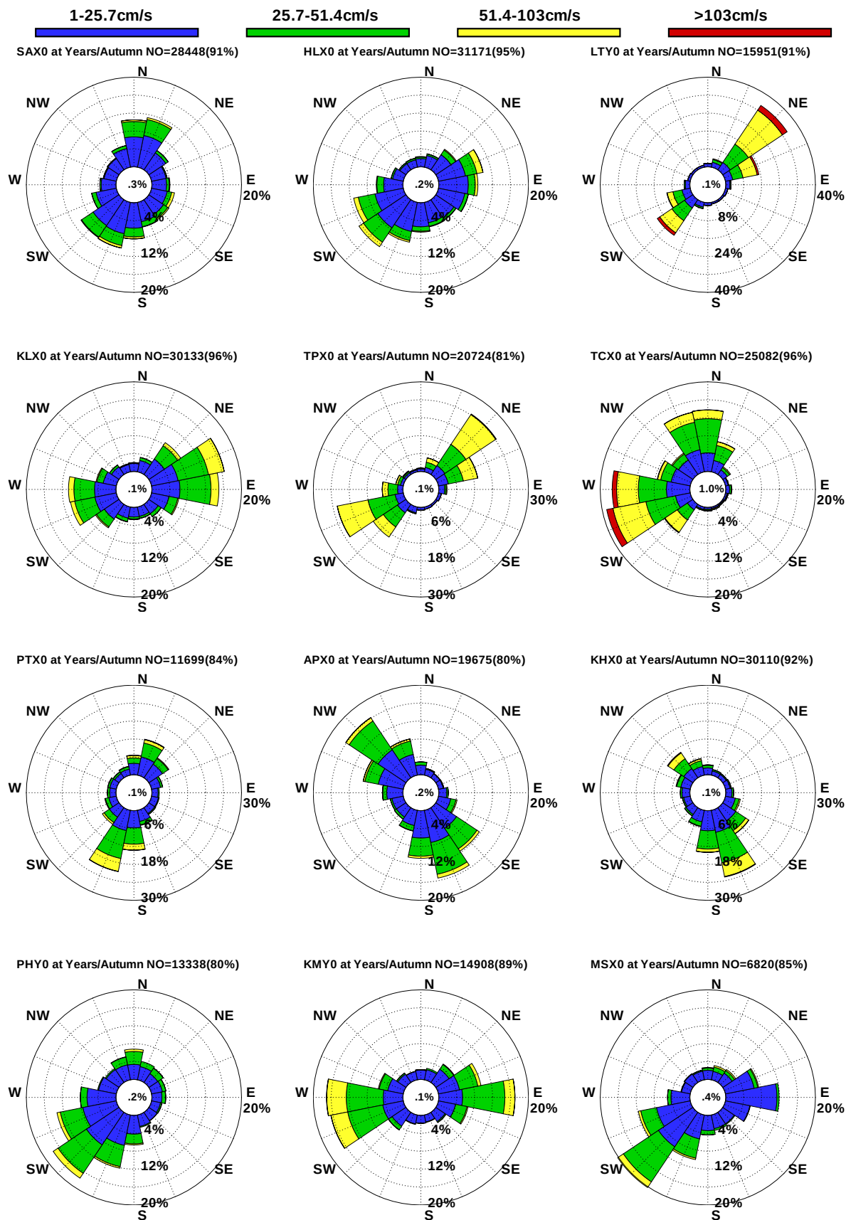
圖9.32 12港域歷年秋季觀測海流玫瑰比較圖
