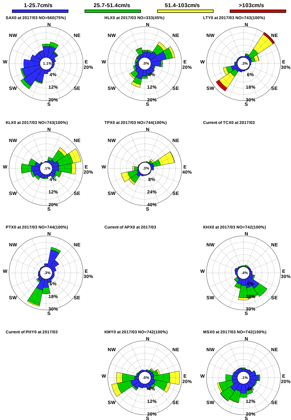
圖9.7 12港域2017年 3月觀測海流玫瑰比較圖
