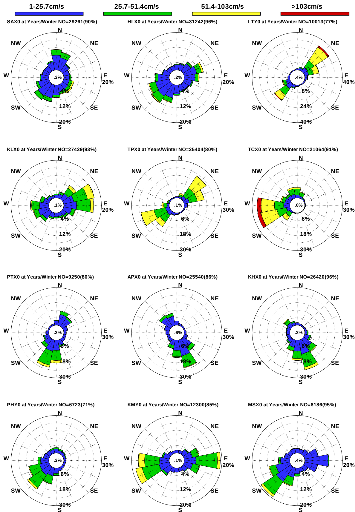
圖9.26 12港域歷年冬季觀測海流玫瑰比較圖
