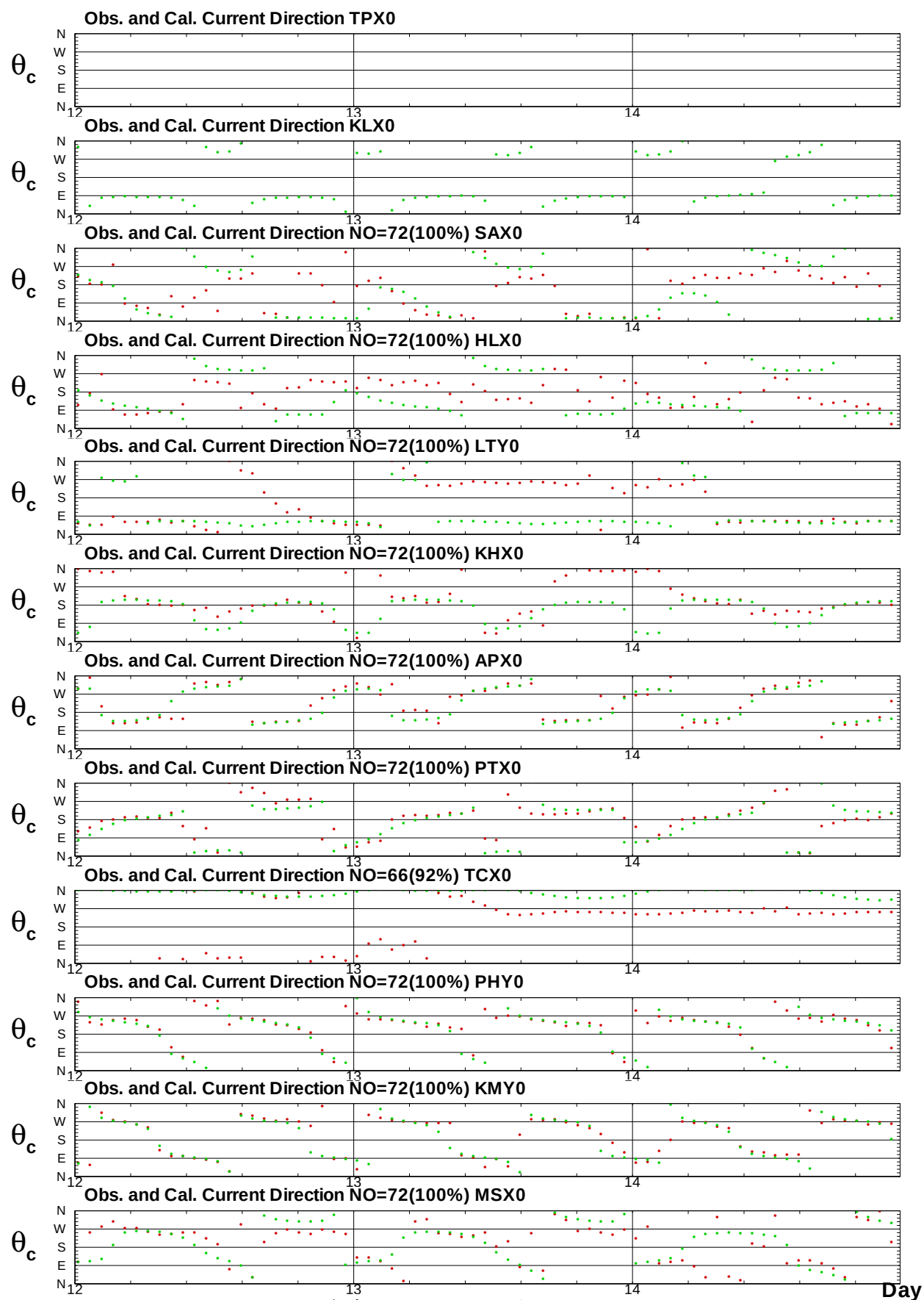
圖10.10 2017年泰利 颱風12海域觀測流向歷線圖 (綠色: 潮流)
