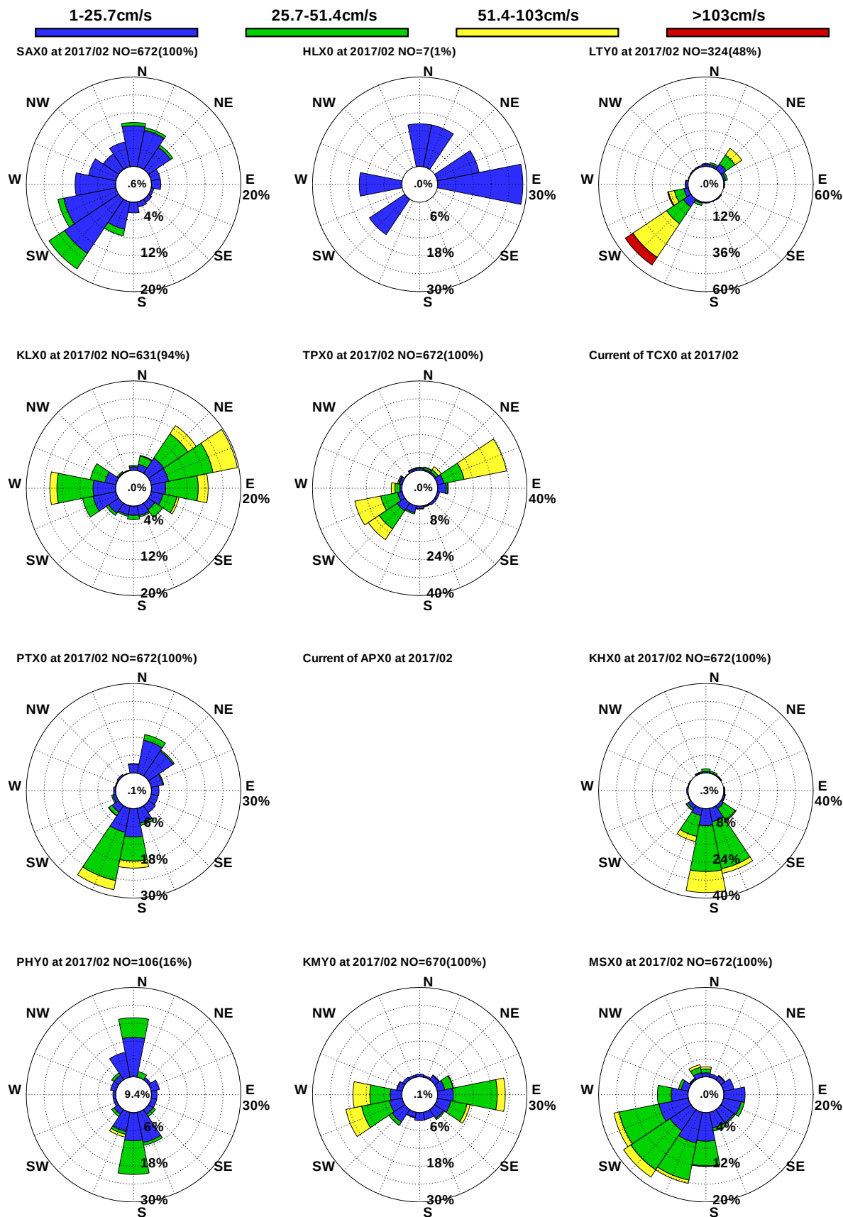
圖9.5 12港域2017年 2月觀測海流玫瑰比較圖
