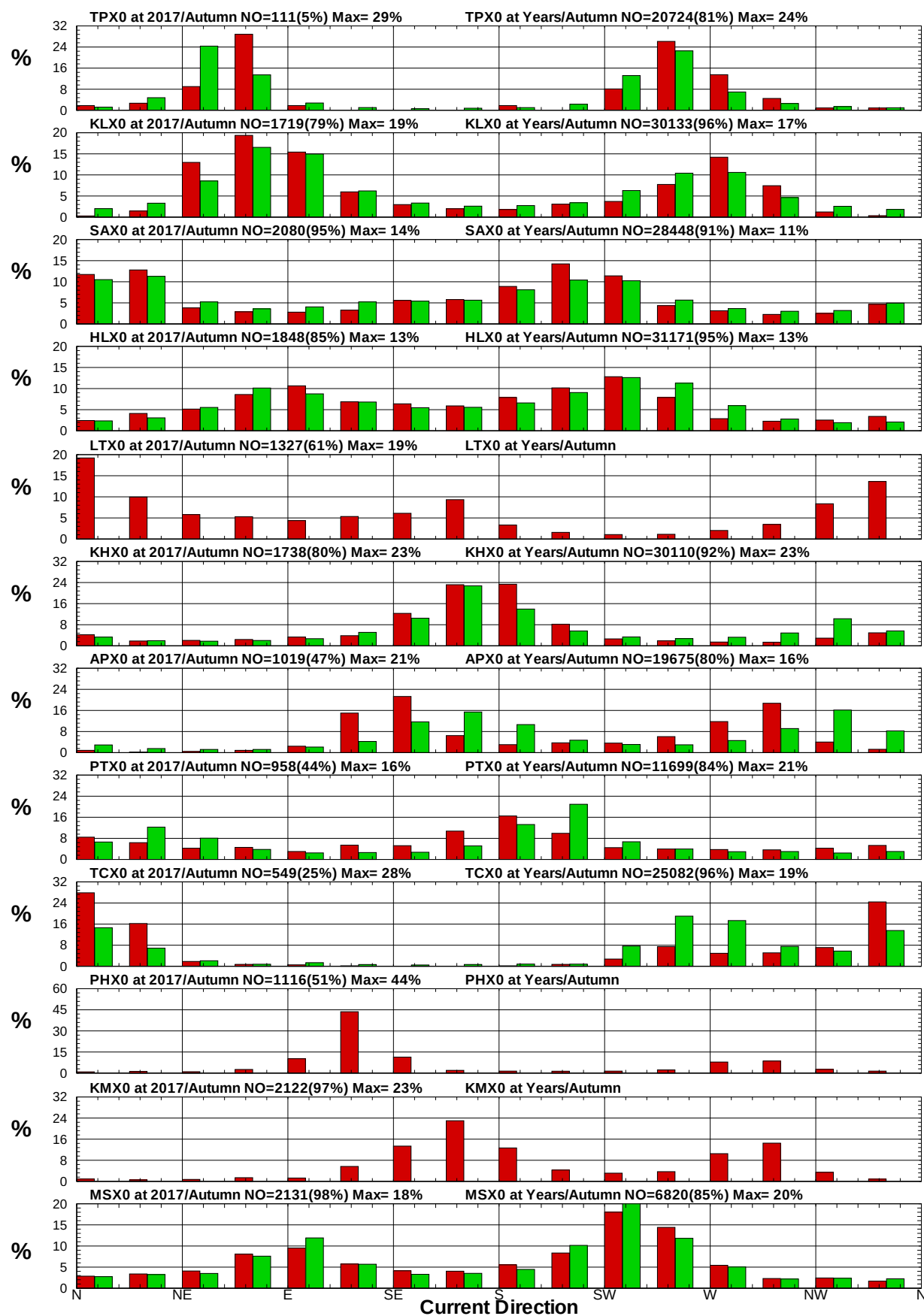
圖8.32 12港域2017年及歷年秋季流向統計方塊圖
