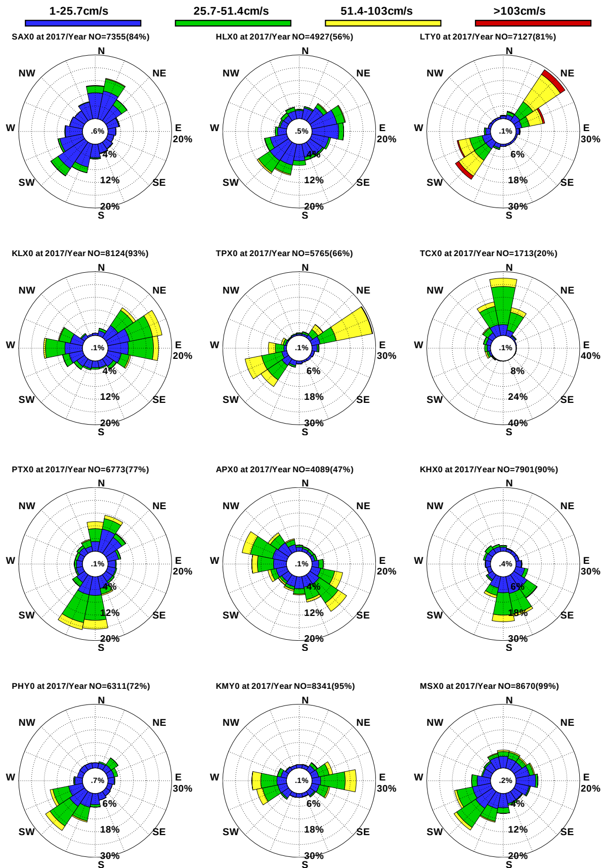
圖9.33 12港域2017年整年觀測海流玫瑰比較圖
