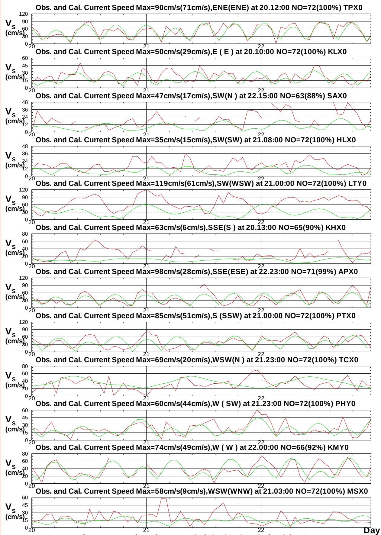
圖10.5 2017年天鵝 颱風12海域觀測流速歷線圖 (綠色: 潮流)
