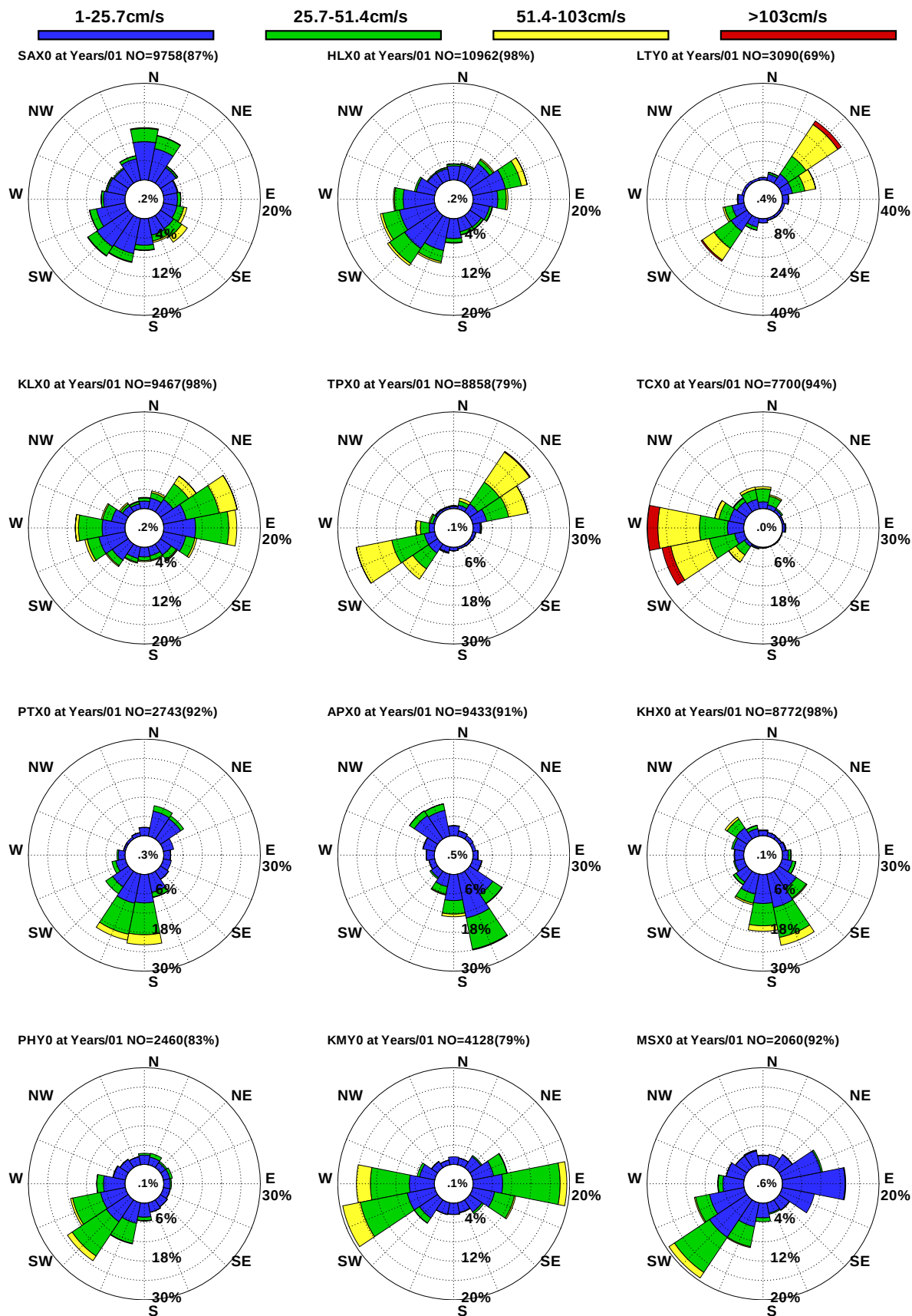
圖9.4 12港域歷年 1 月觀測海流玫瑰比較圖
