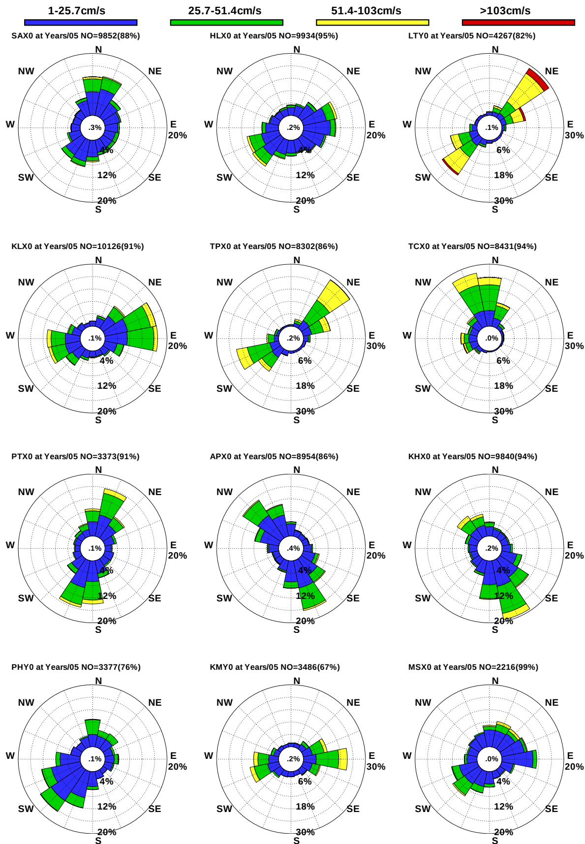
圖9.12 12港域歷年 5 月觀測海流玫瑰比較圖
