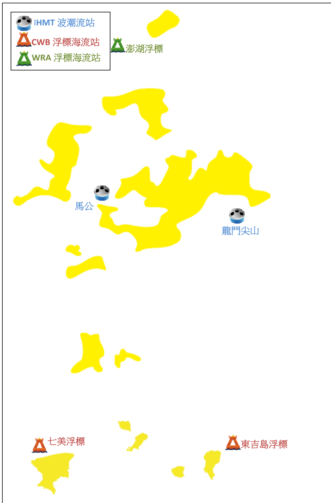
圖 1.10 澎湖海域海流觀測站位置示意圖
