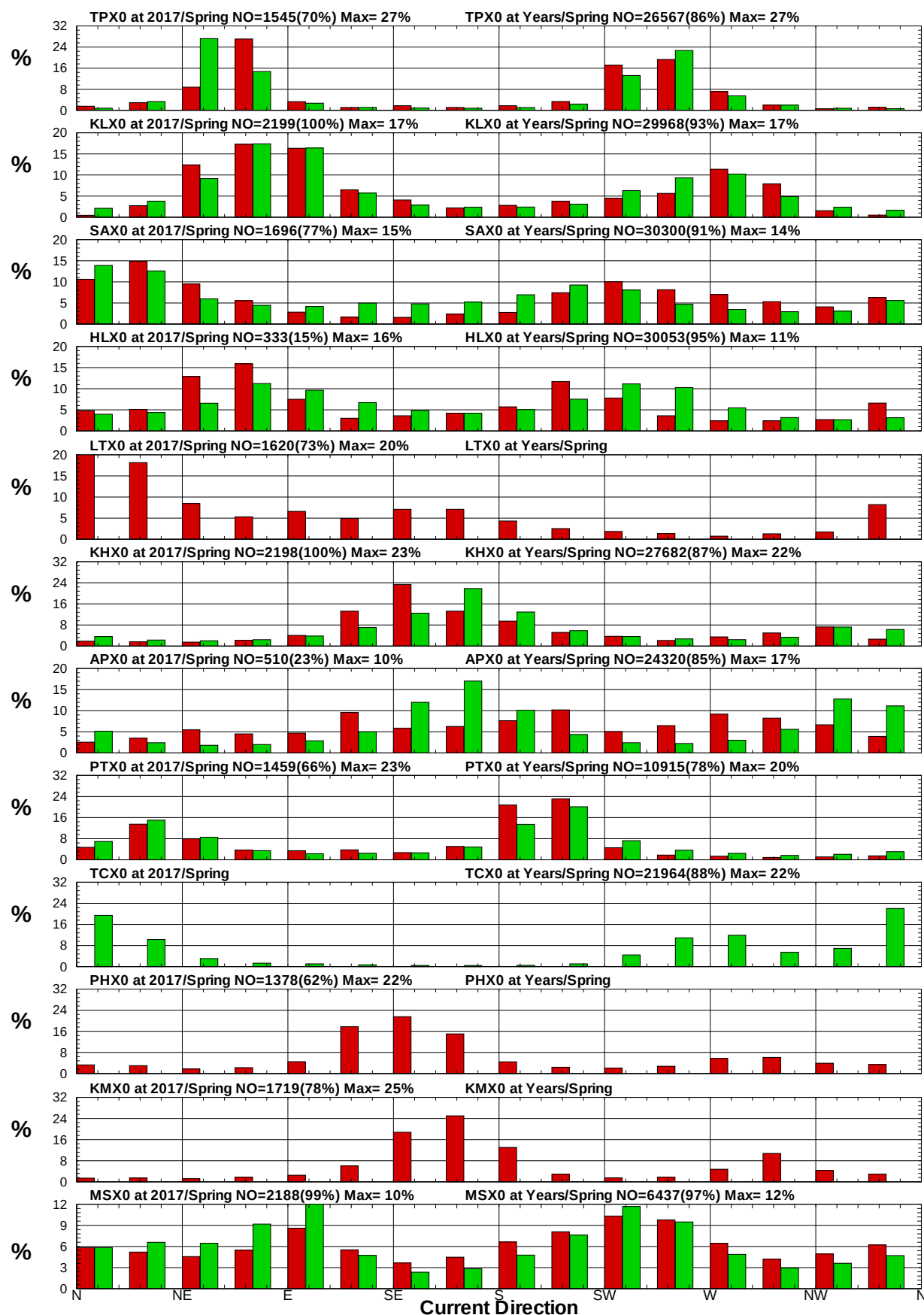
圖8.28 12港域2017年及歷年春季流向統計方塊圖
