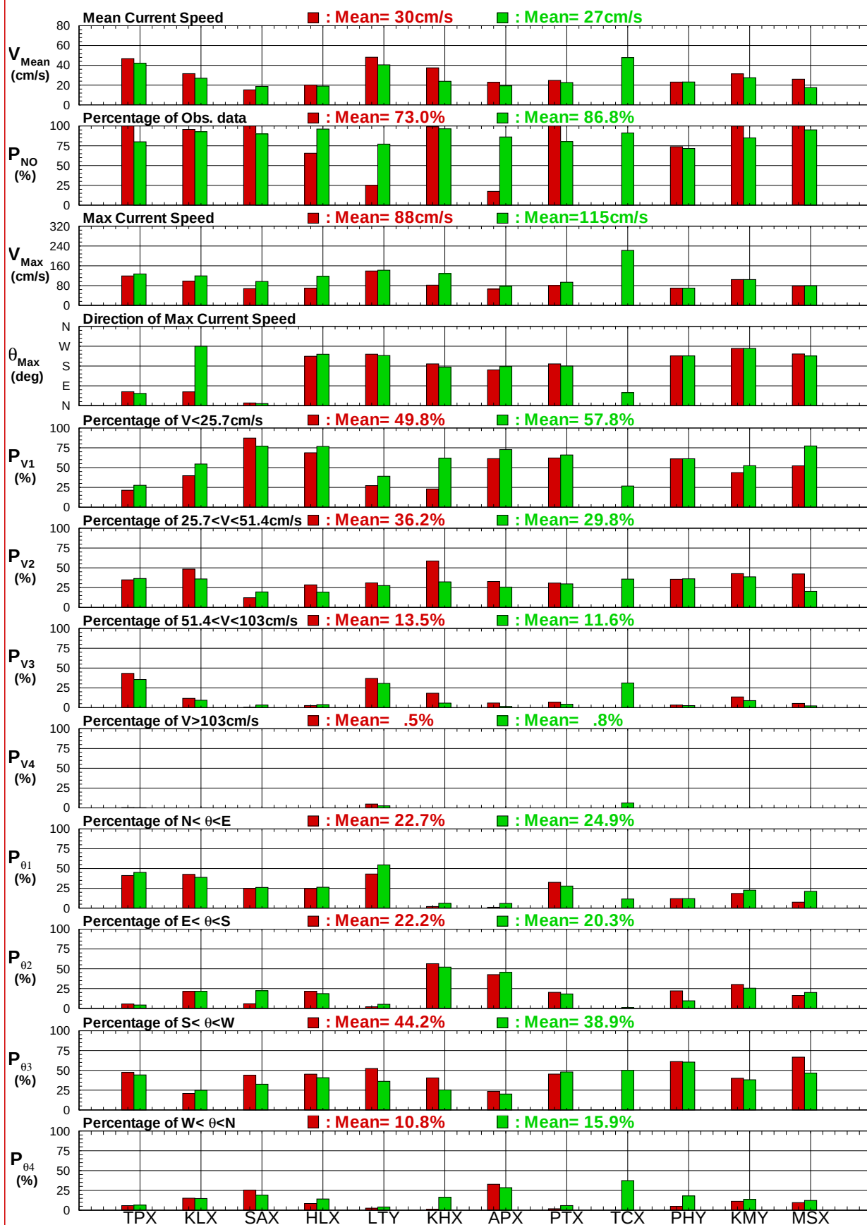
圖7.1a 12個港域2017及歷年主要測站冬季流速(向)比較圖
