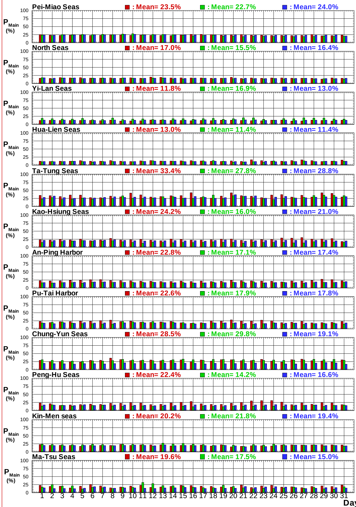
圖7.7f 歷年12港域冬, 夏及整年主要測站每日主要流向百分比圖
