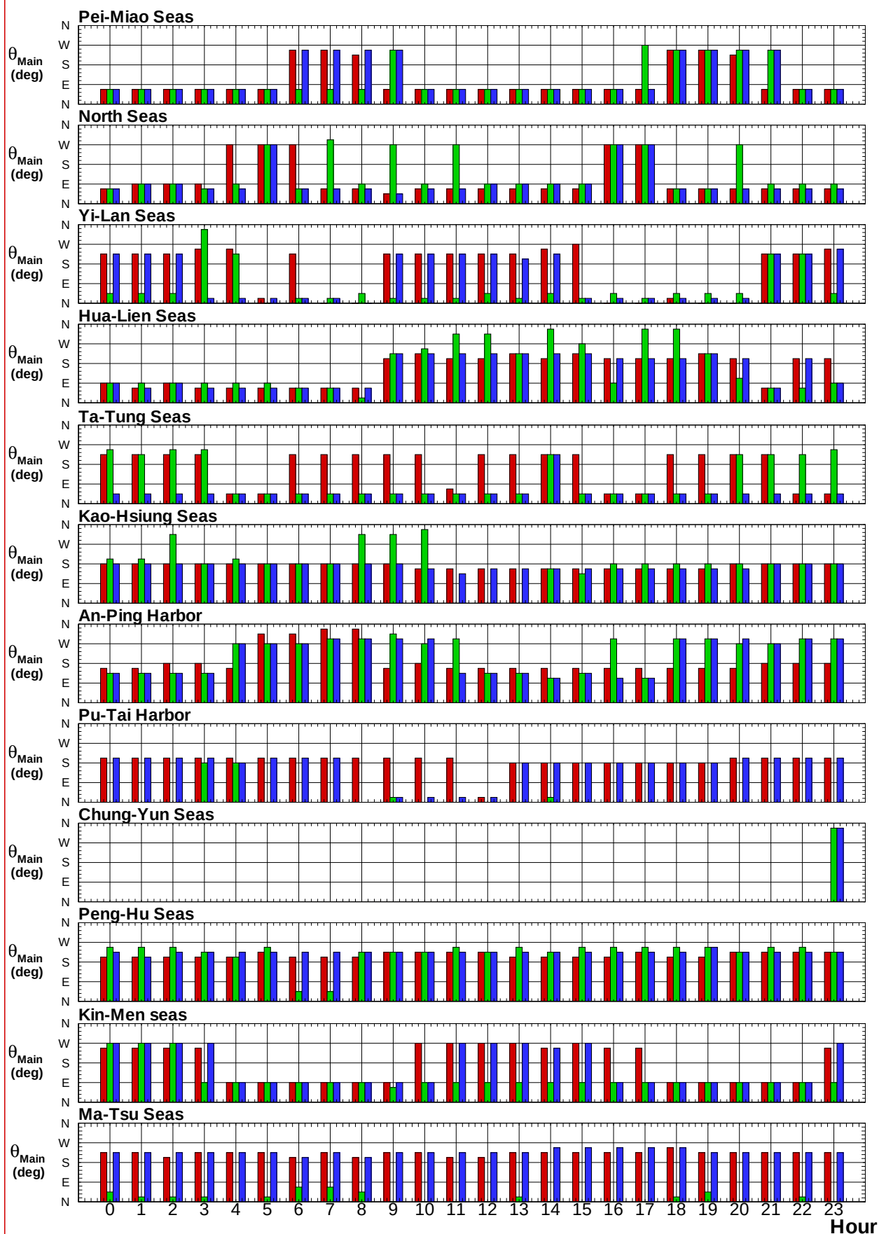
圖7.4e 2017年12港域冬, 夏及整年主要測站逐時主要流向比較圖
