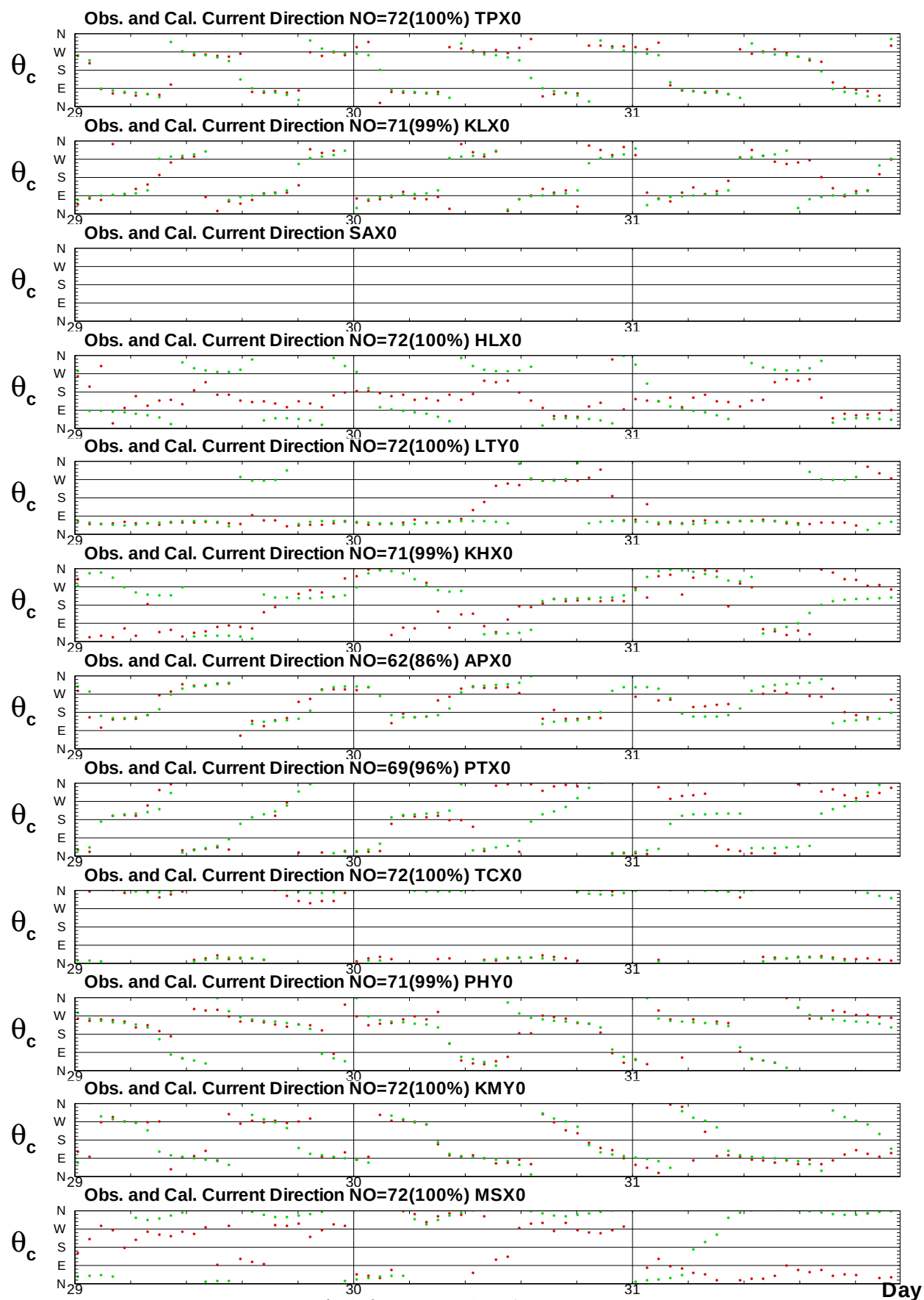
圖10.4 2017年海棠 颱風12海域觀測流向歷線圖 (綠色: 潮流)
