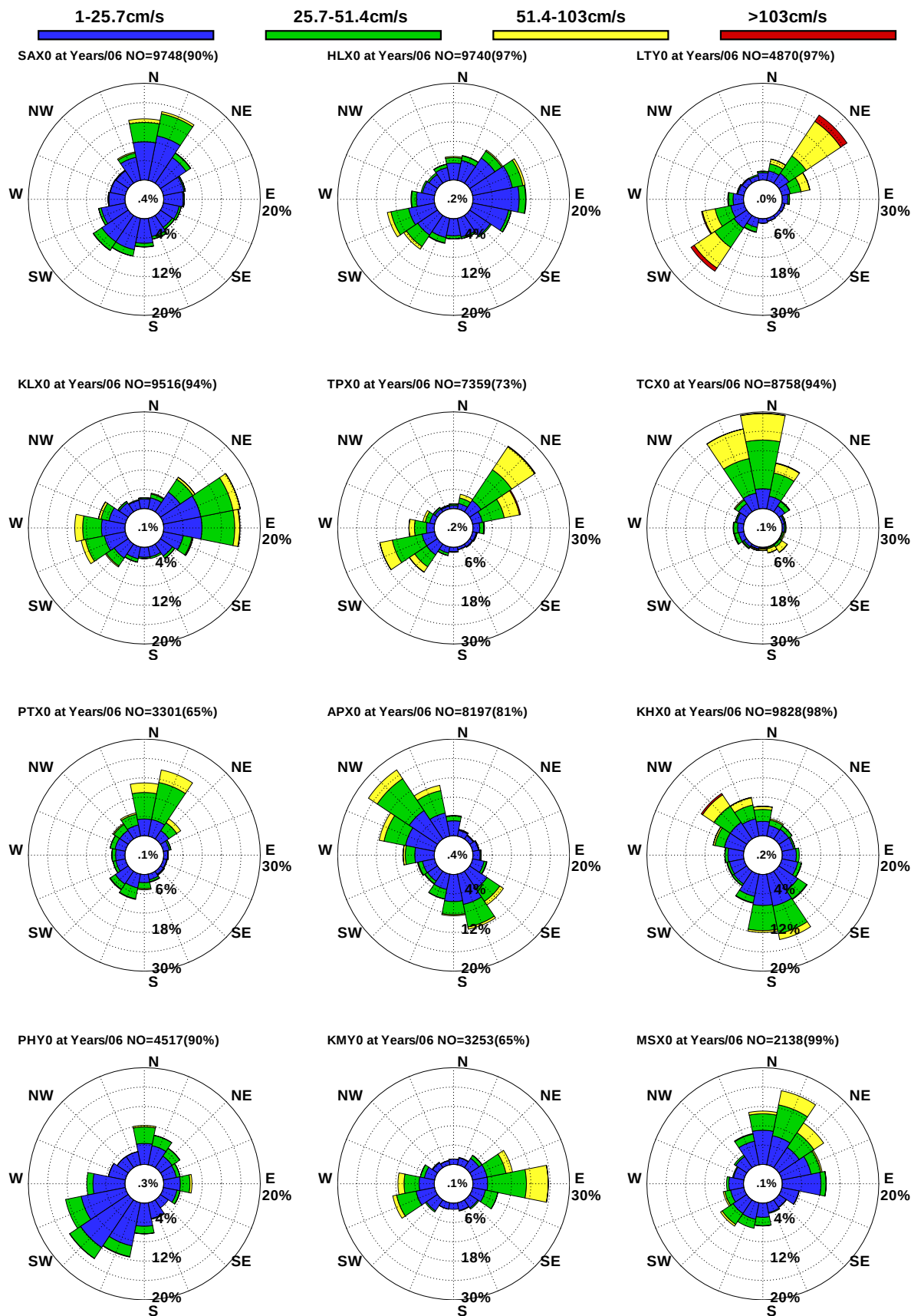
圖9.14 12港域歷年 6 月觀測海流玫瑰比較圖
