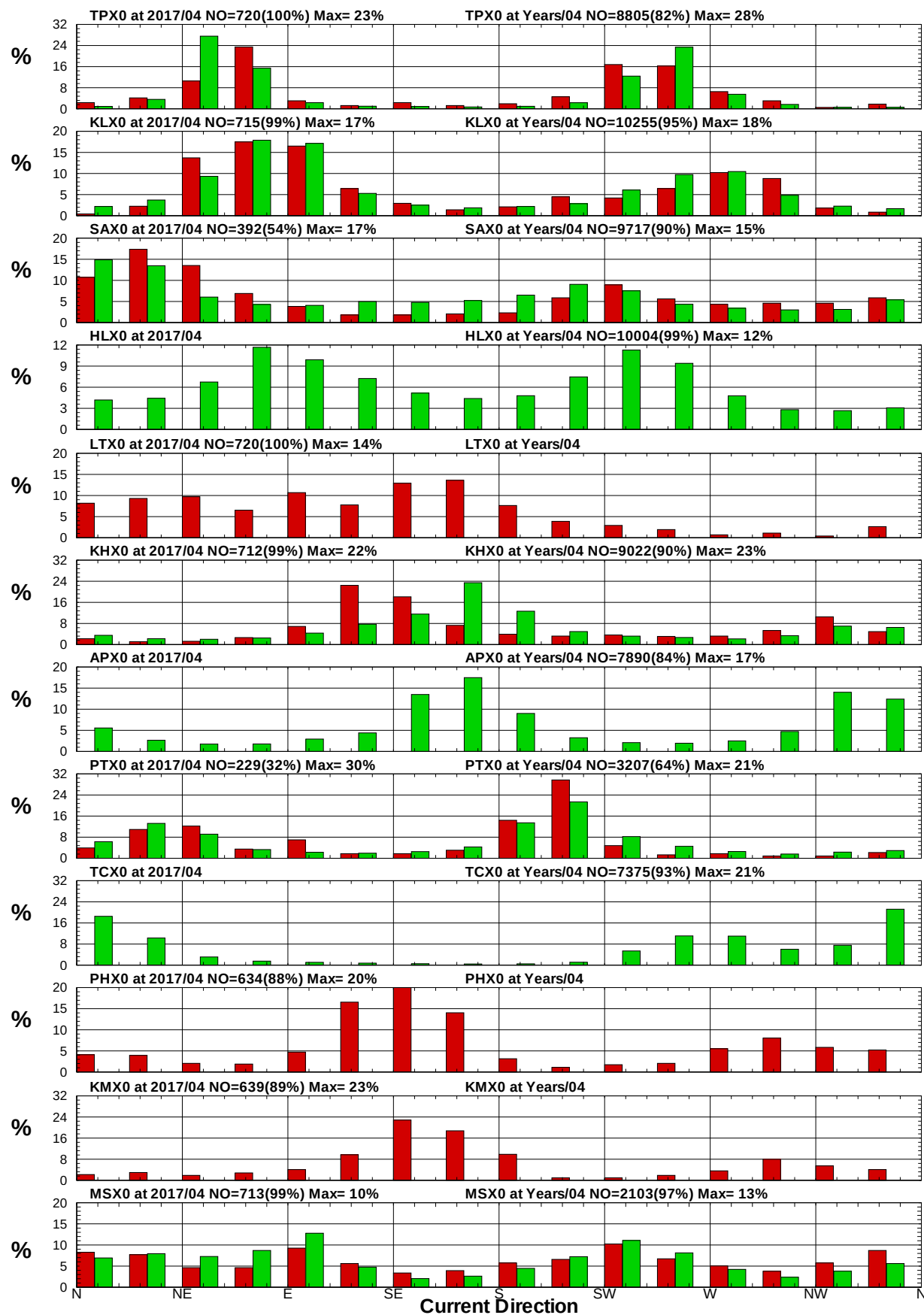
圖8.10 12港域2017年及歷年 4月流向統計方塊圖
