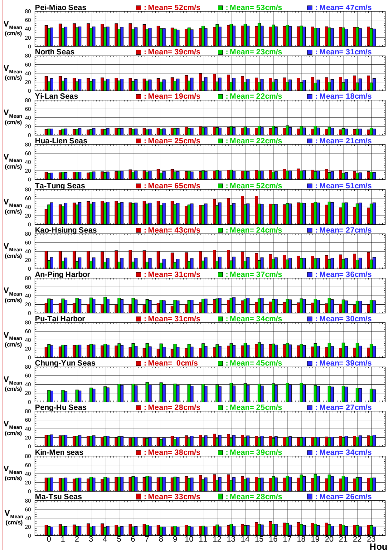
圖7.4a 2017年12港域冬, 夏及整年主要測站逐時平均流速比較圖
