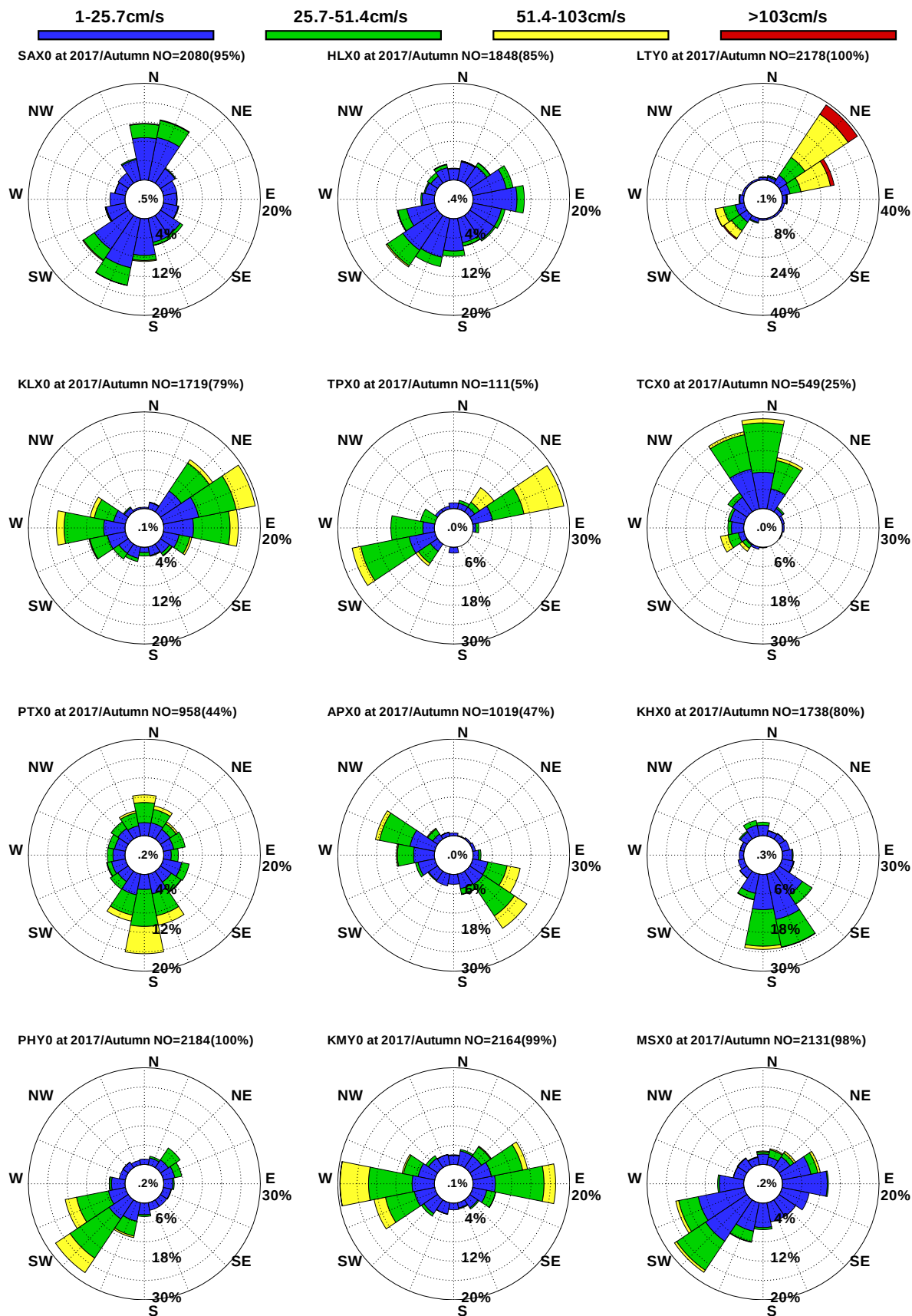
圖9.31 12港域2017年秋季觀測海流玫瑰比較圖
