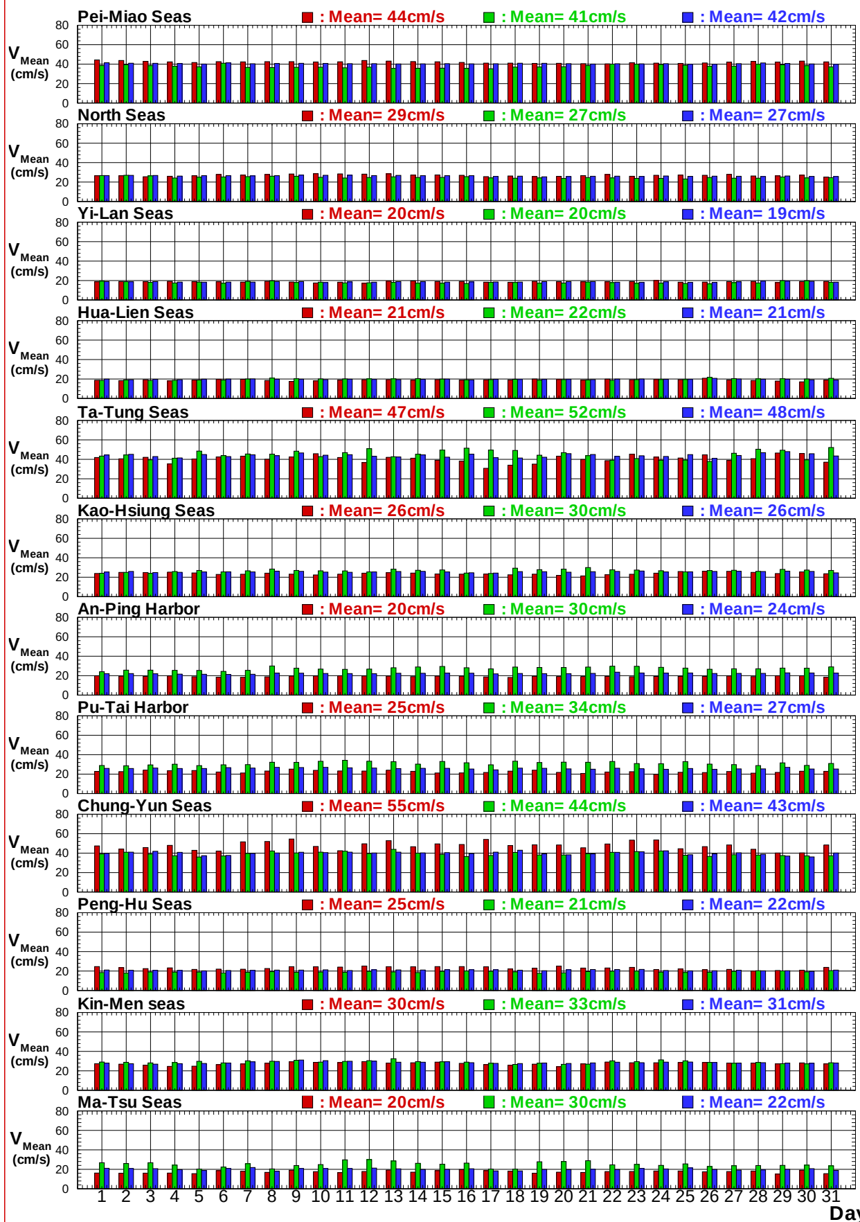
圖7.7a 歷年12港域冬, 夏及整年主要測站每日平均流速比較圖
