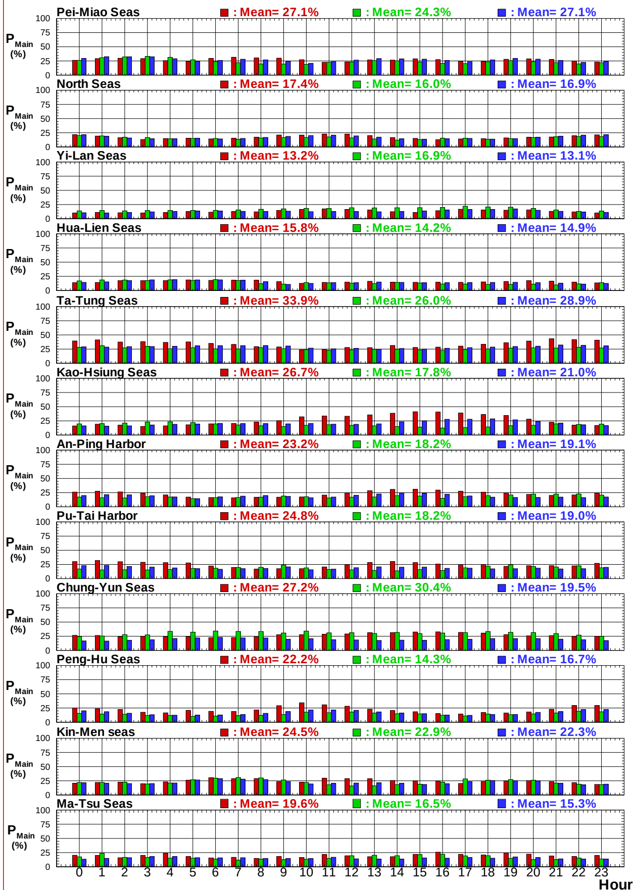
圖7.5f 歷年12港域冬, 夏及整年主要測站逐時主要流向百分比圖
