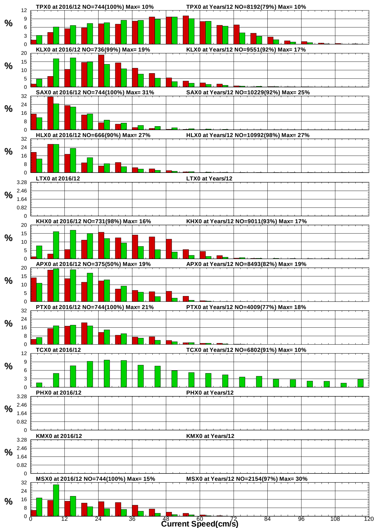
圖8.1 12港域2016年及歷年12月流速統計方塊圖
