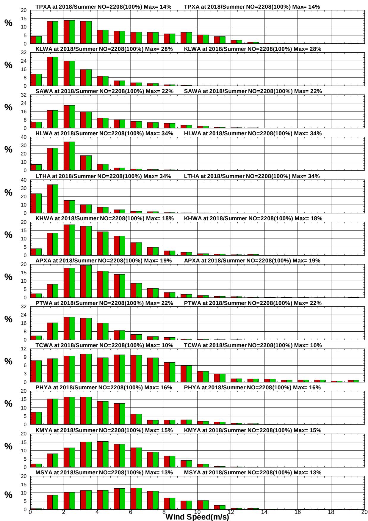
圖9.29 12港域2018年夏季年12月風速統計方塊圖
