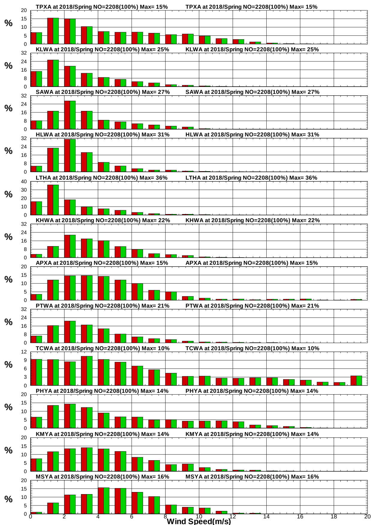
圖9.27 12港域2018年春季年12月風速統計方塊圖
