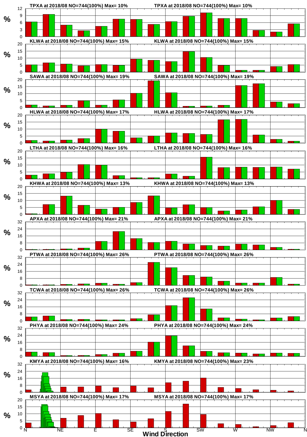
圖9.18 12港域2018年8月12月風向統計方塊圖
