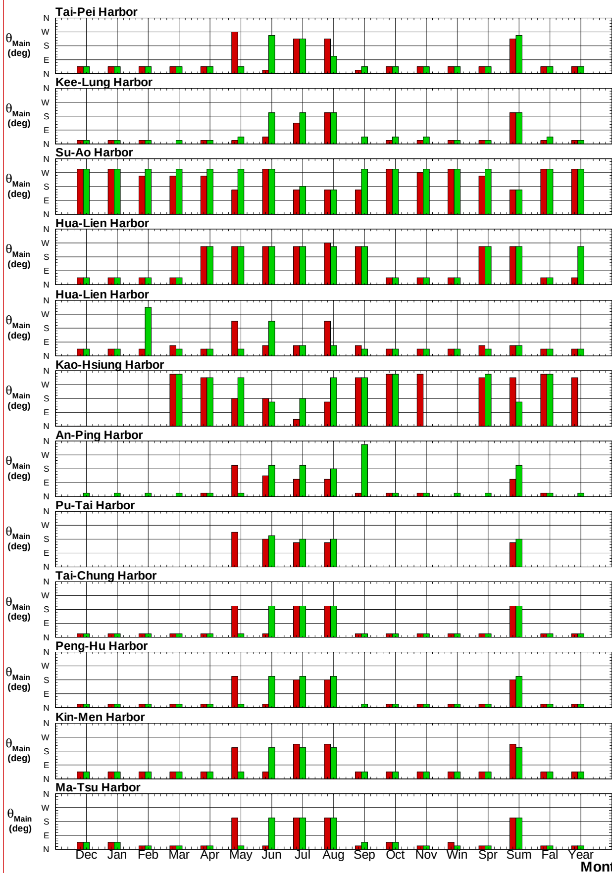
圖8.3e 2018及歷年12港域主要測站每月(季)主要風向比較圖
