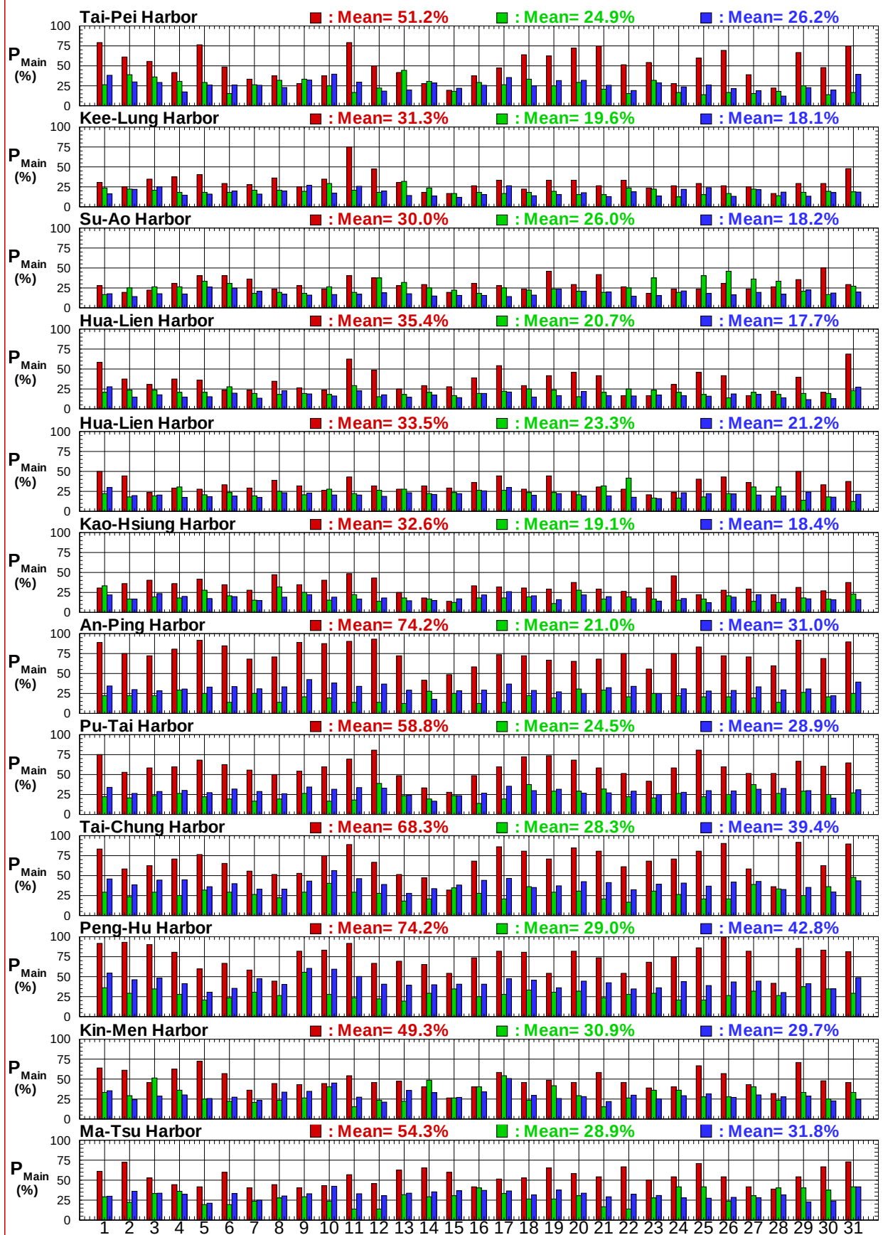
圖8.6f 2018年12港域冬, 夏及整年主要測站每日主要風向百分比圖
