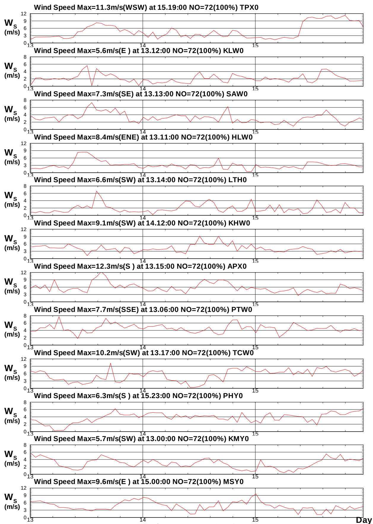
圖11.3 2018年山竹 颱風12海域觀測風速歷線圖
