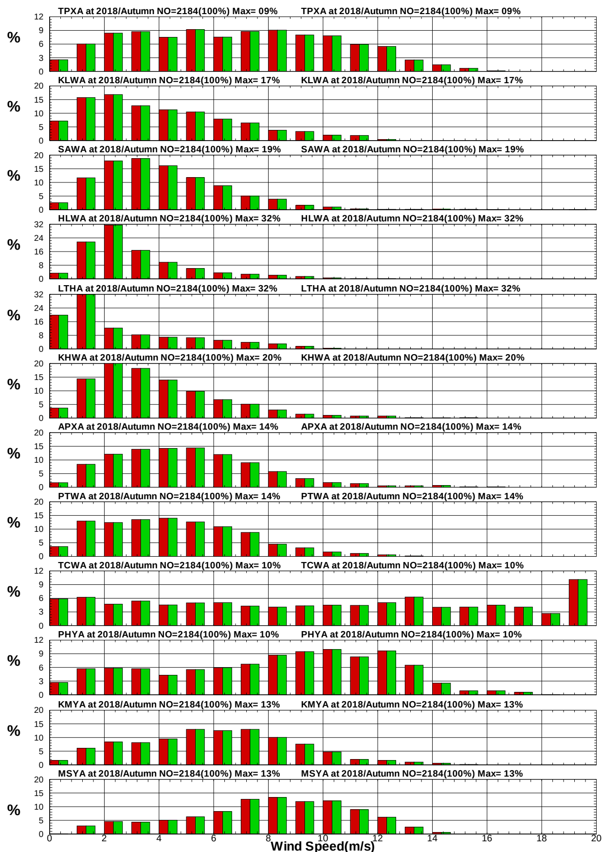
圖9.31 12港域2018年秋季年12月風速統計方塊圖
