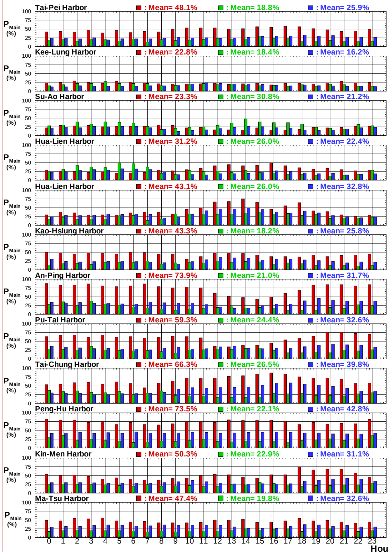
圖8.4f 2018年12港域冬, 夏及整年主要測站逐時主要風向百分比圖
