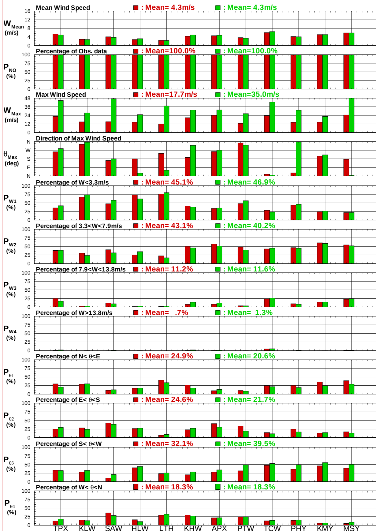
圖8.1c 12個港域2018及歷年主要測站夏季風速(向)比較圖
