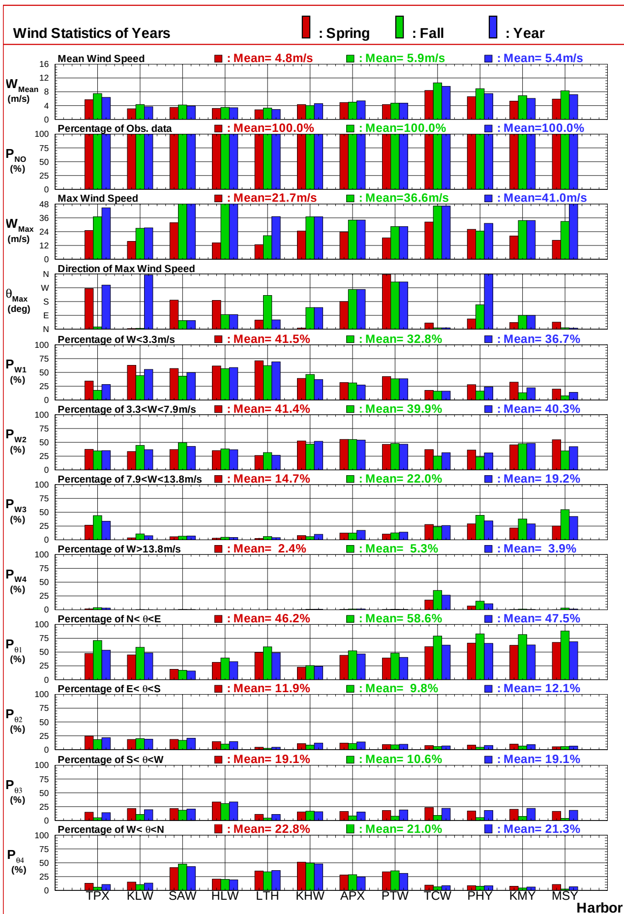
圖8.2d 12個港域歷年主要測站春, 秋及整年風速 (向) 比較圖
