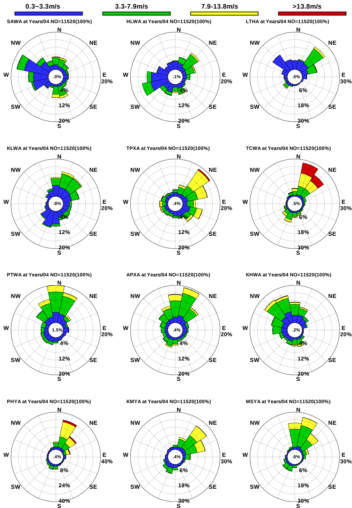
圖10.10 12港域歷年 4 月觀測風玫瑰比較圖
