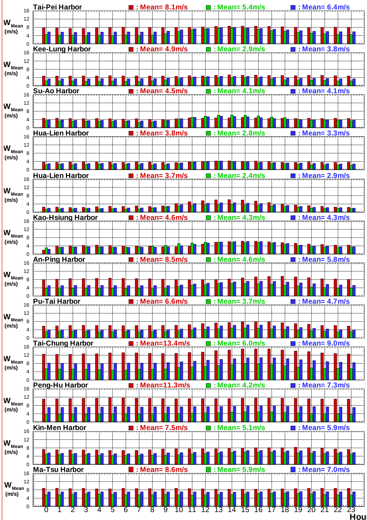
圖8.4a 2018年12港域冬、夏及整年主要測站逐時平均風速比較圖
