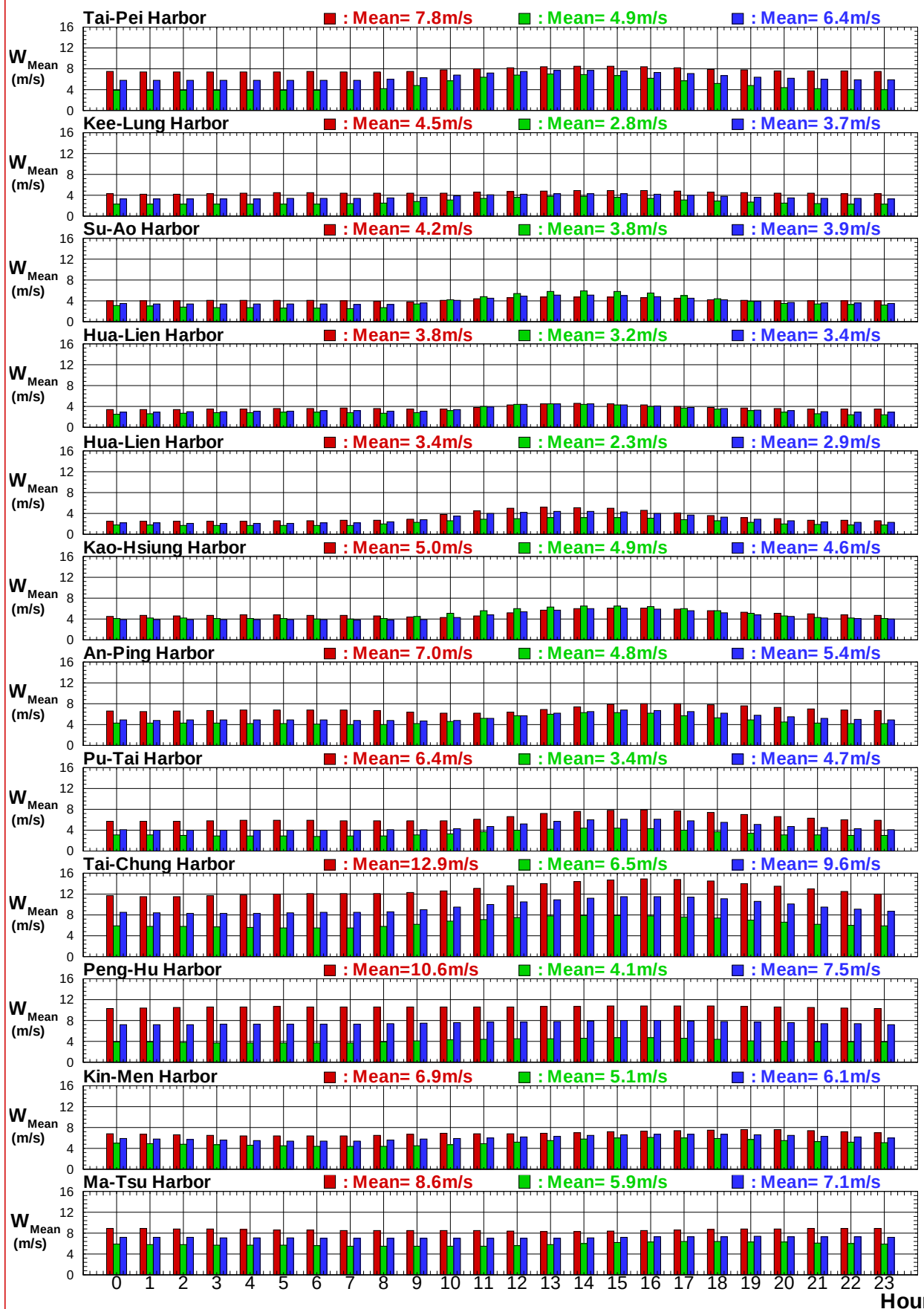
圖8.5a 歷年12港域冬, 夏及整年主要測站逐時平均風速比較圖
