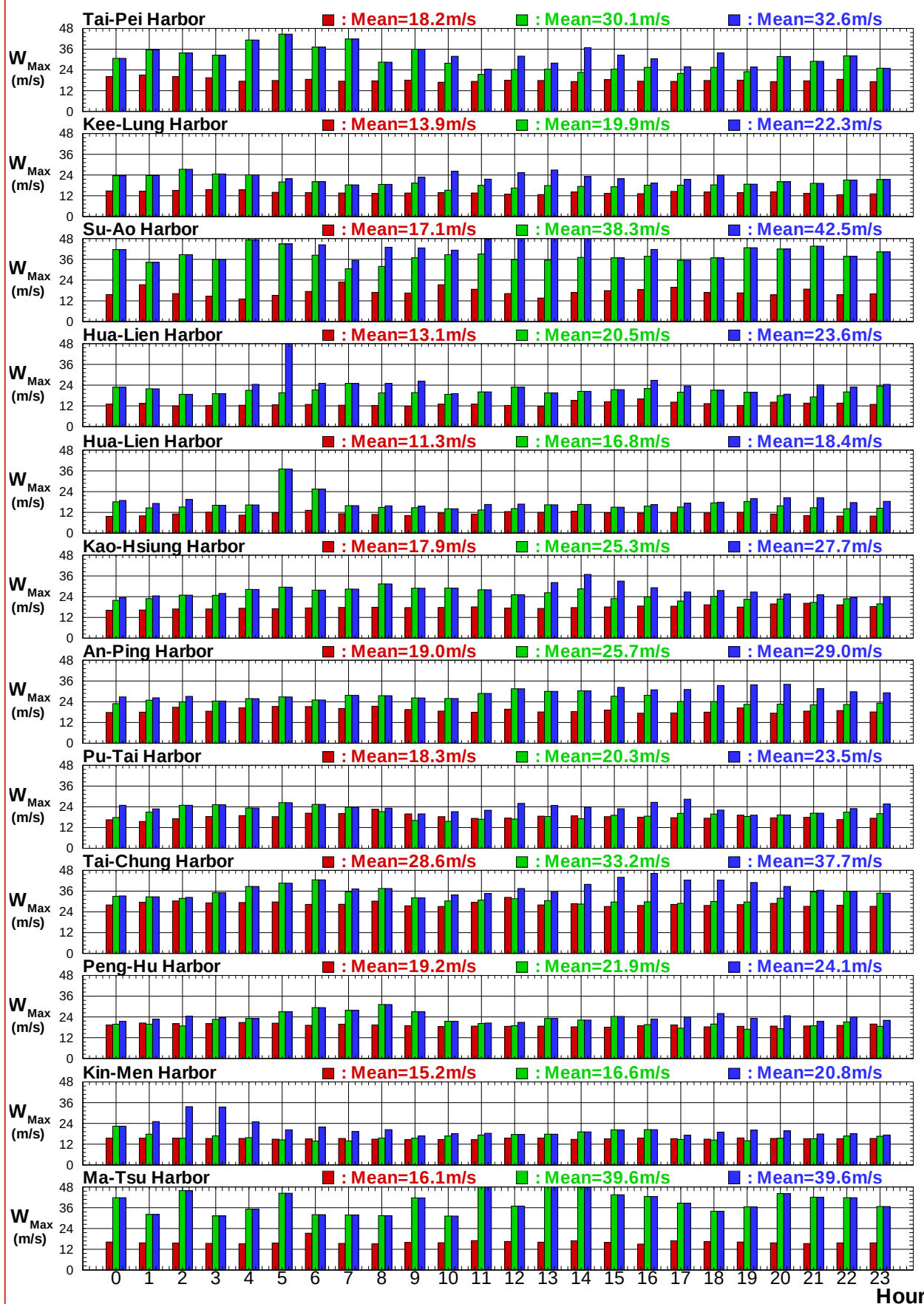
圖8.5c 歷年12港域冬, 夏及整年主要測站逐時最大風速比較圖
