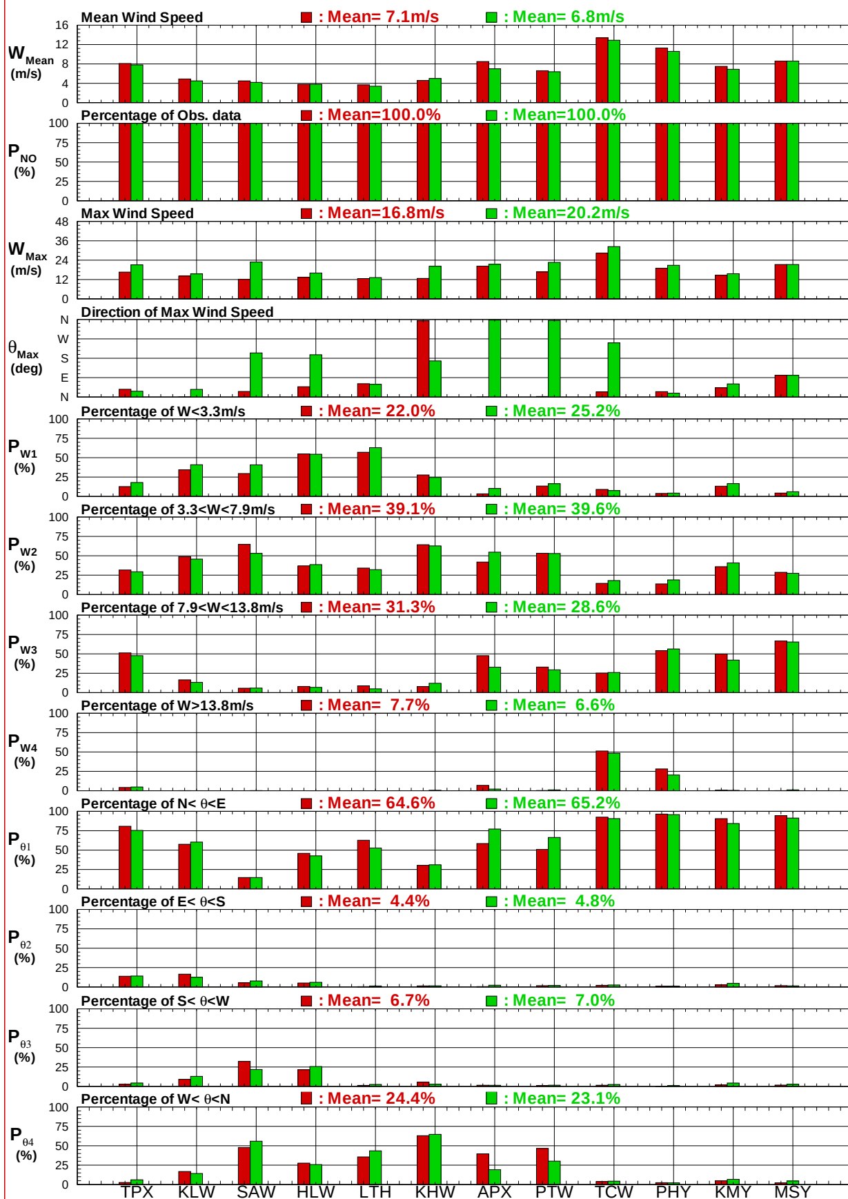
圖8.1a 12個港域2018及歷年主要測站冬季風速(向)比較圖
