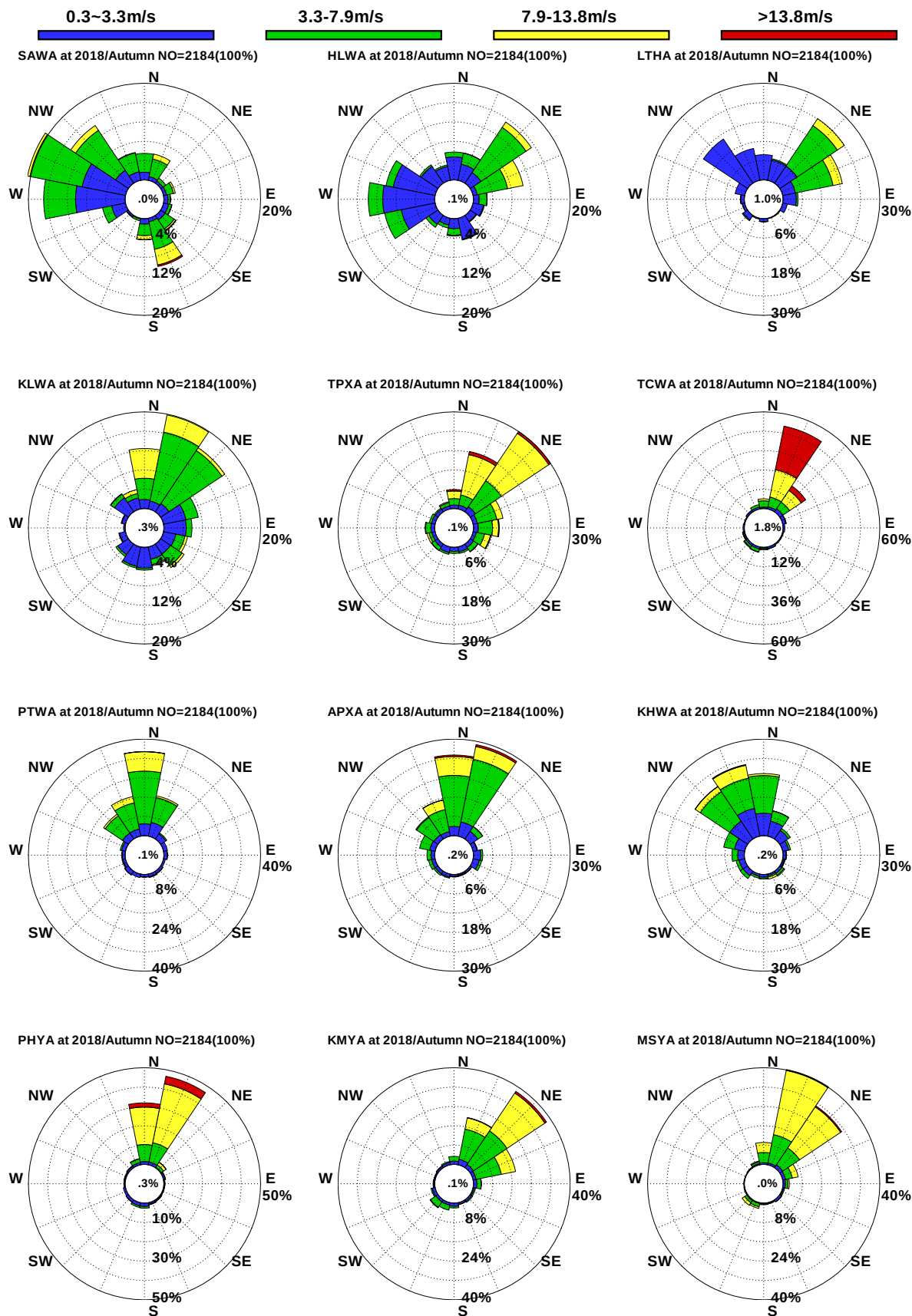
圖10.31 12港域2018年秋季觀測風玫瑰比較圖
