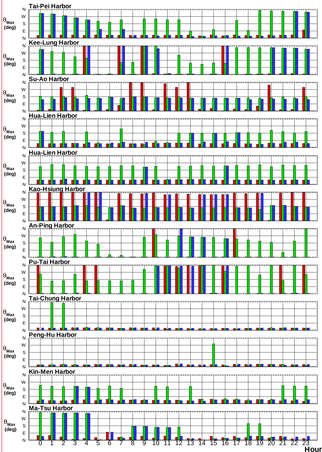
圖8.4d 2018年12港域冬, 夏及整年主要測站逐時最大風速之風向圖
