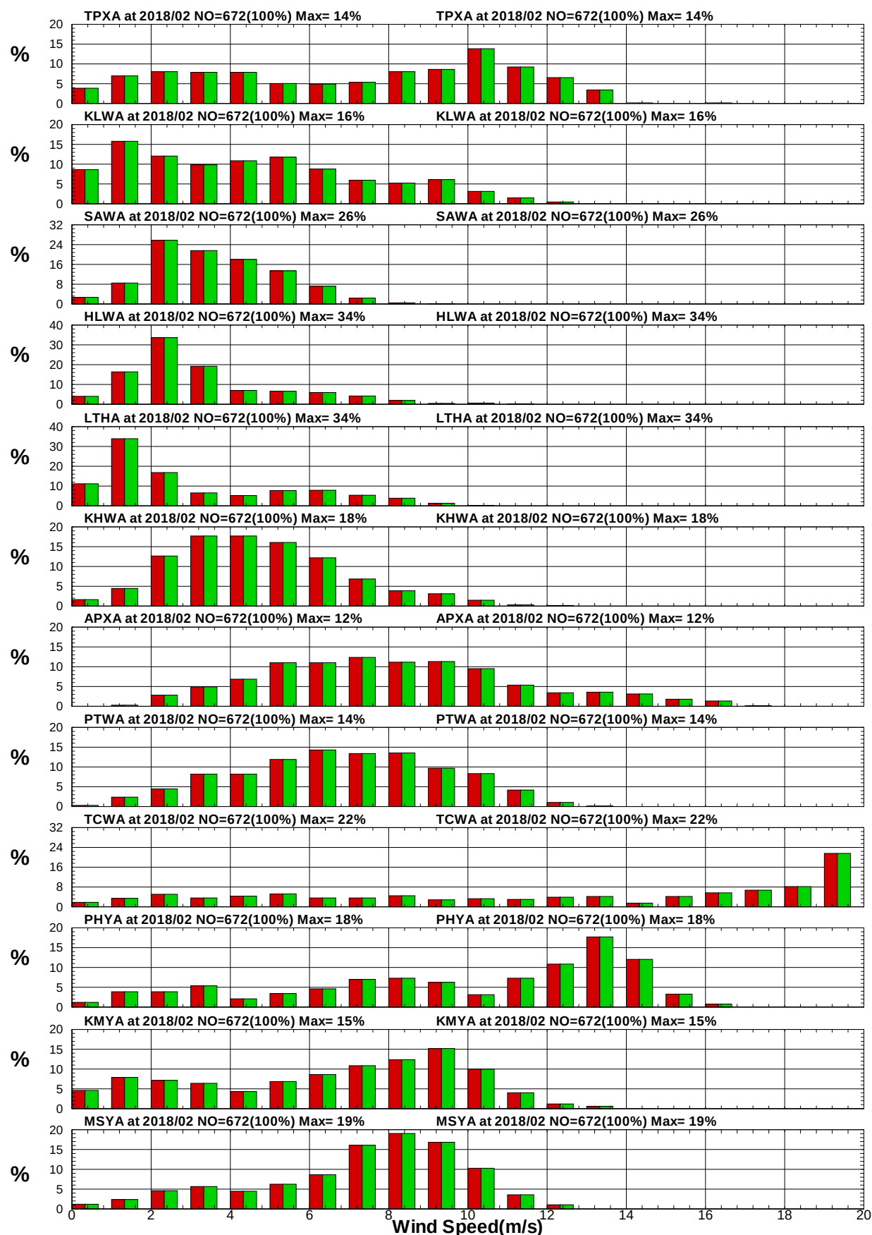
圖9.5 12港域2018年 2月年12月風速統計方塊圖
