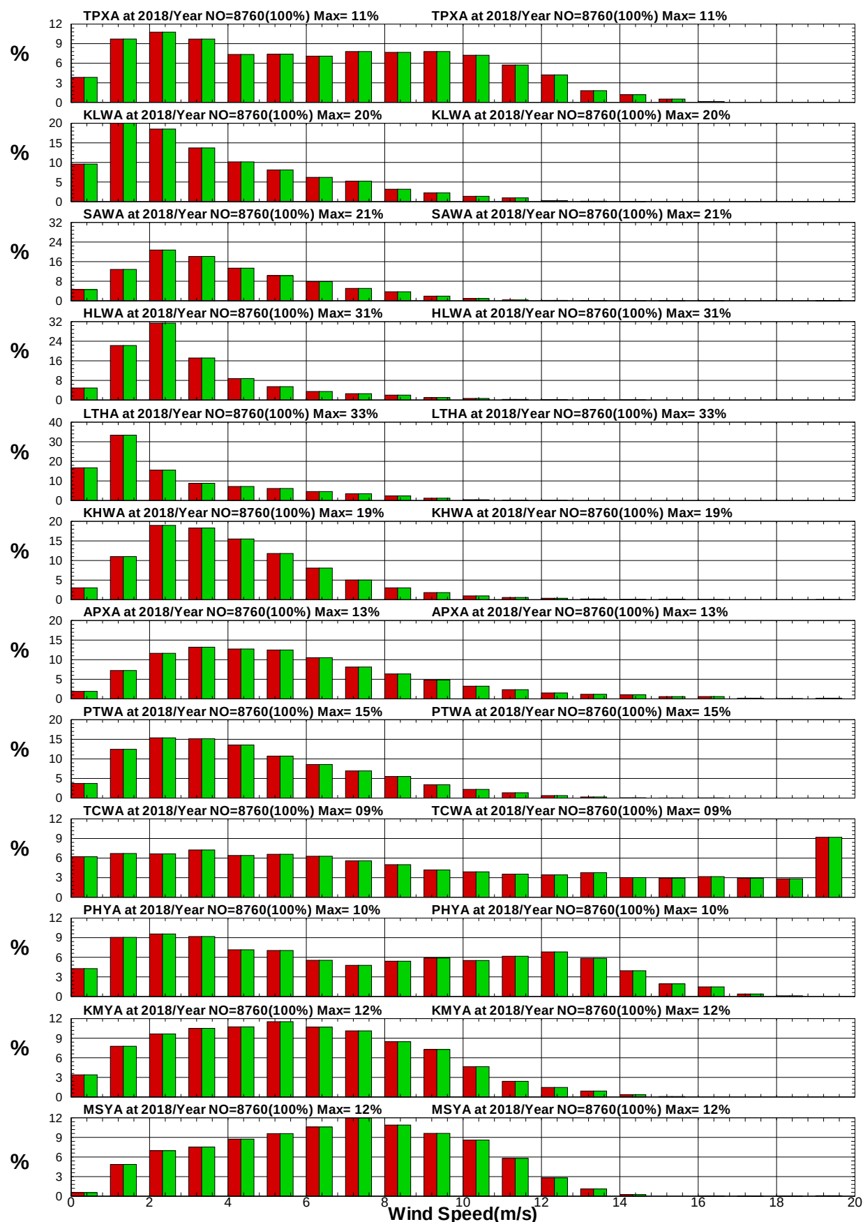
圖9.33 12港域2018年整年年12月風速統計方塊圖
