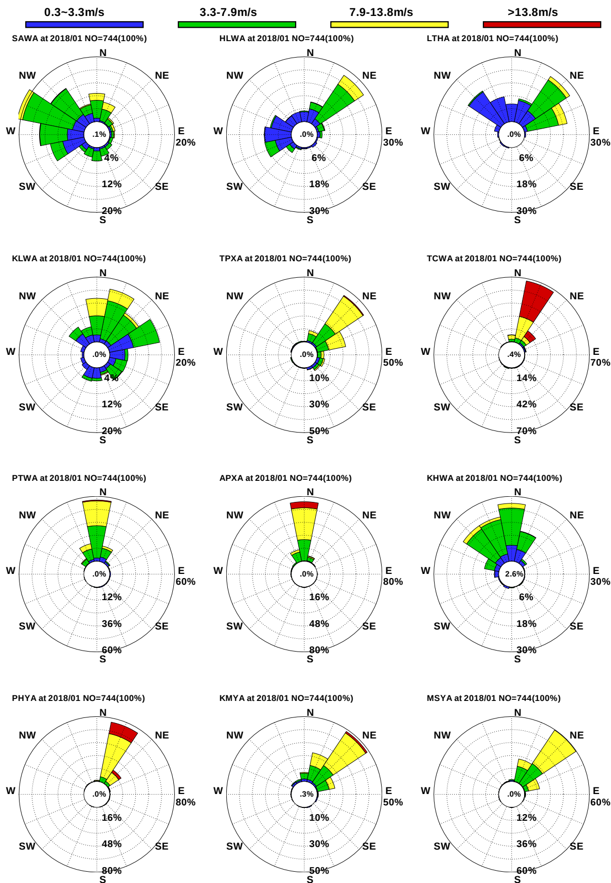
圖10.3 12港域2018年 1月觀測風玫瑰比較圖
