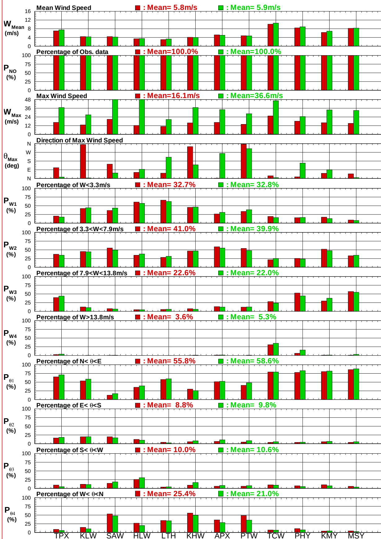
圖8.1d 12個港域2018及歷年主要測站秋季風速 (向) 比較圖
