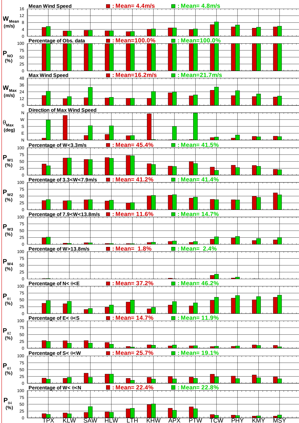
圖8.1b 12個港域2018及歷年主要測站春季風速 (向) 比較圖
