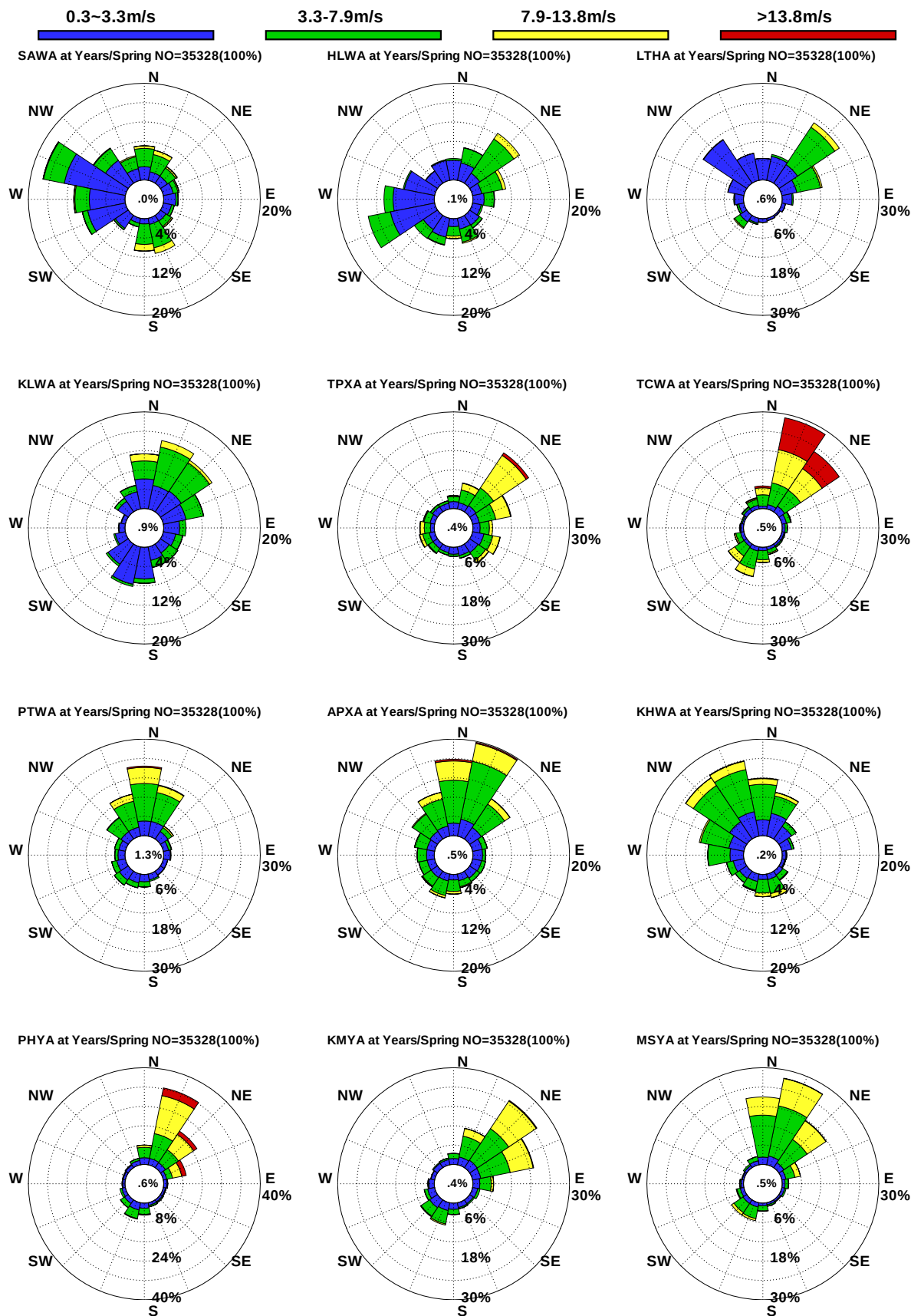
圖10.28 12港域歷年春季觀測風玫瑰比較圖
