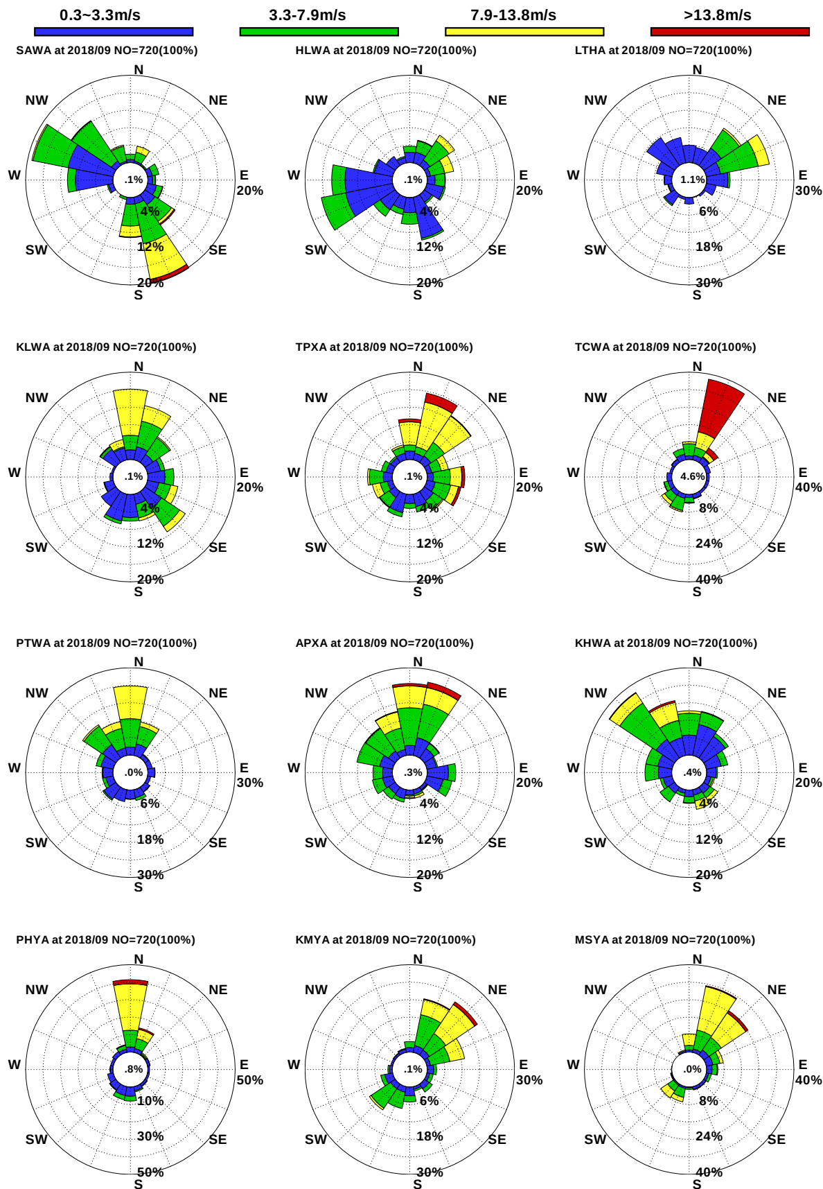
圖10.19 12港域2018年 9月觀測風玫瑰比較圖
