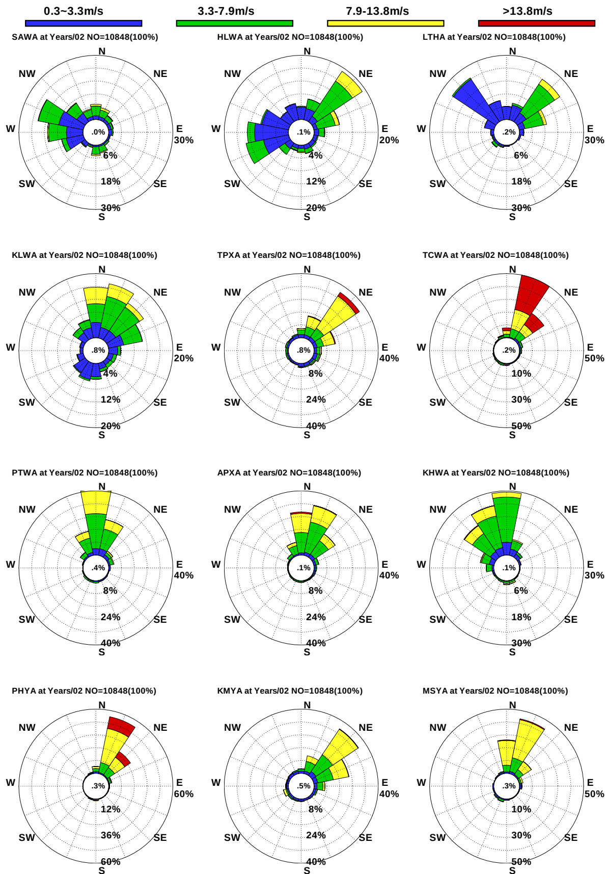
圖10.6 12港域歷年 2月觀測風玫瑰比較圖
