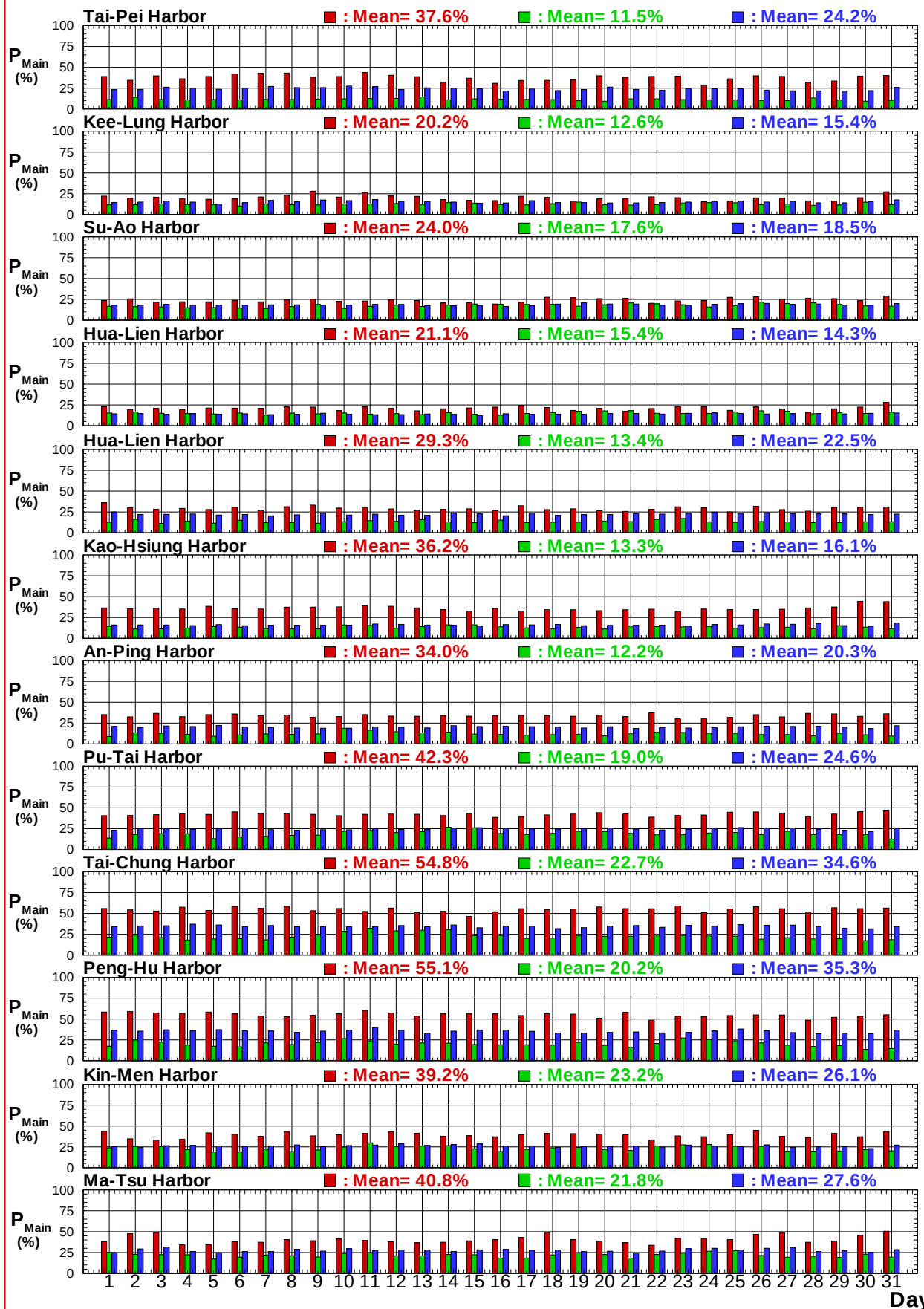
圖8.7f 歷年12港域冬, 夏及整年主要測站每日主要風向百分比圖
