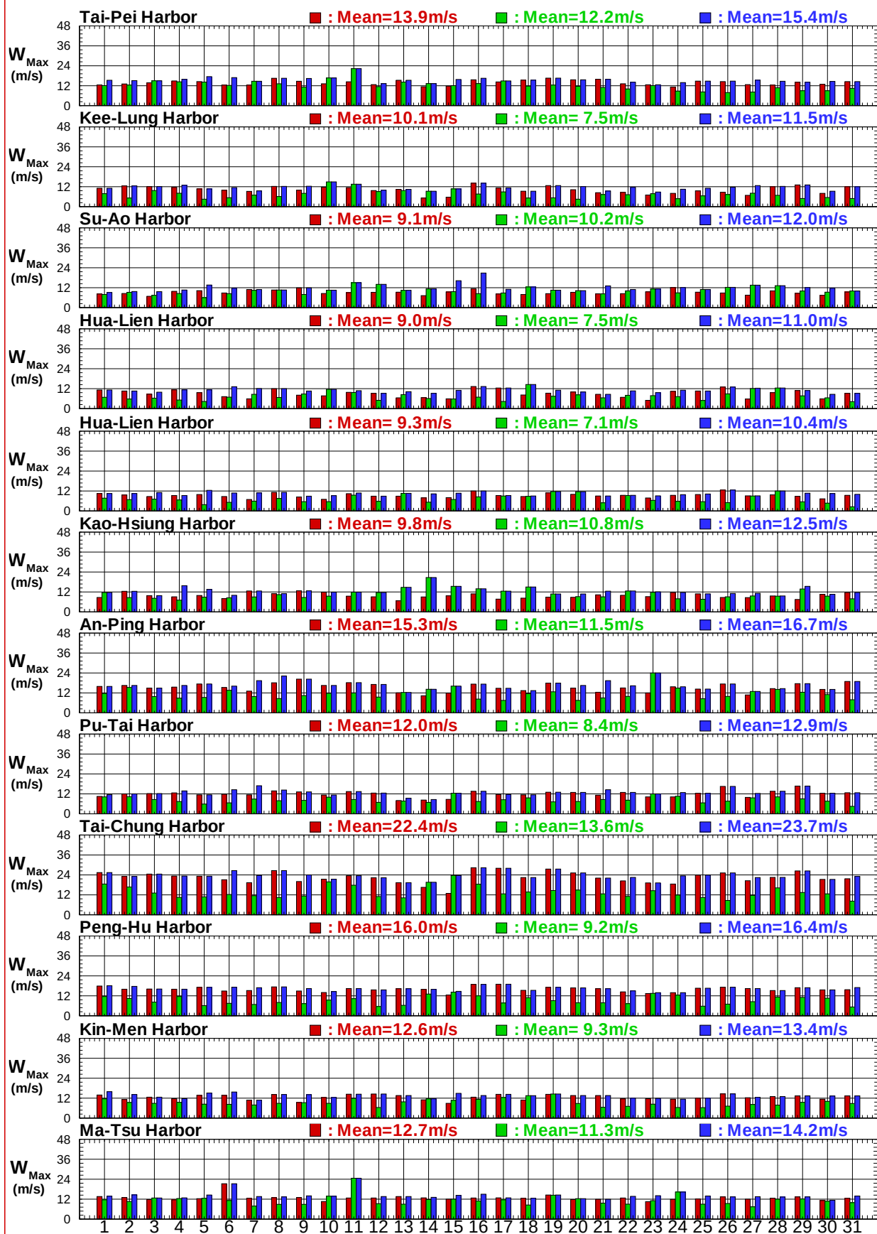
圖8.6c 2018年12港域冬、夏及整年主要測站每日最大風速比較圖
