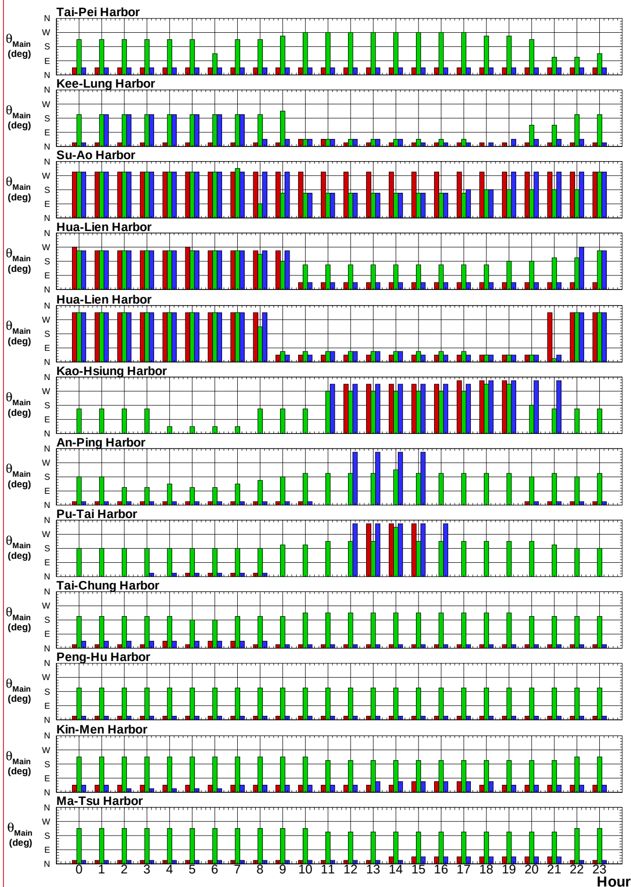
圖8.5e 歷年12港域冬, 夏及整年主要測站逐時主要風向比較圖
