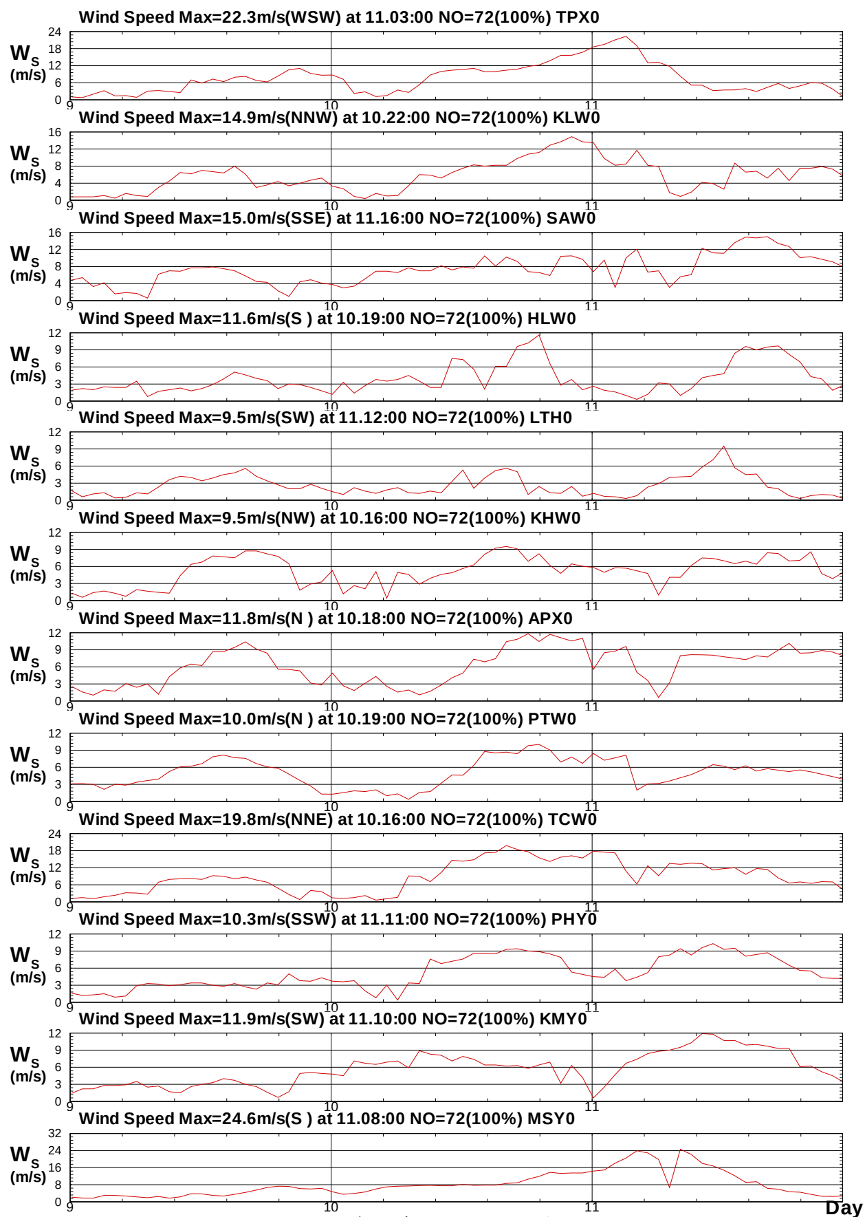
圖11.1 2018年瑪莉亞颱風12海域觀測風速歷線圖
