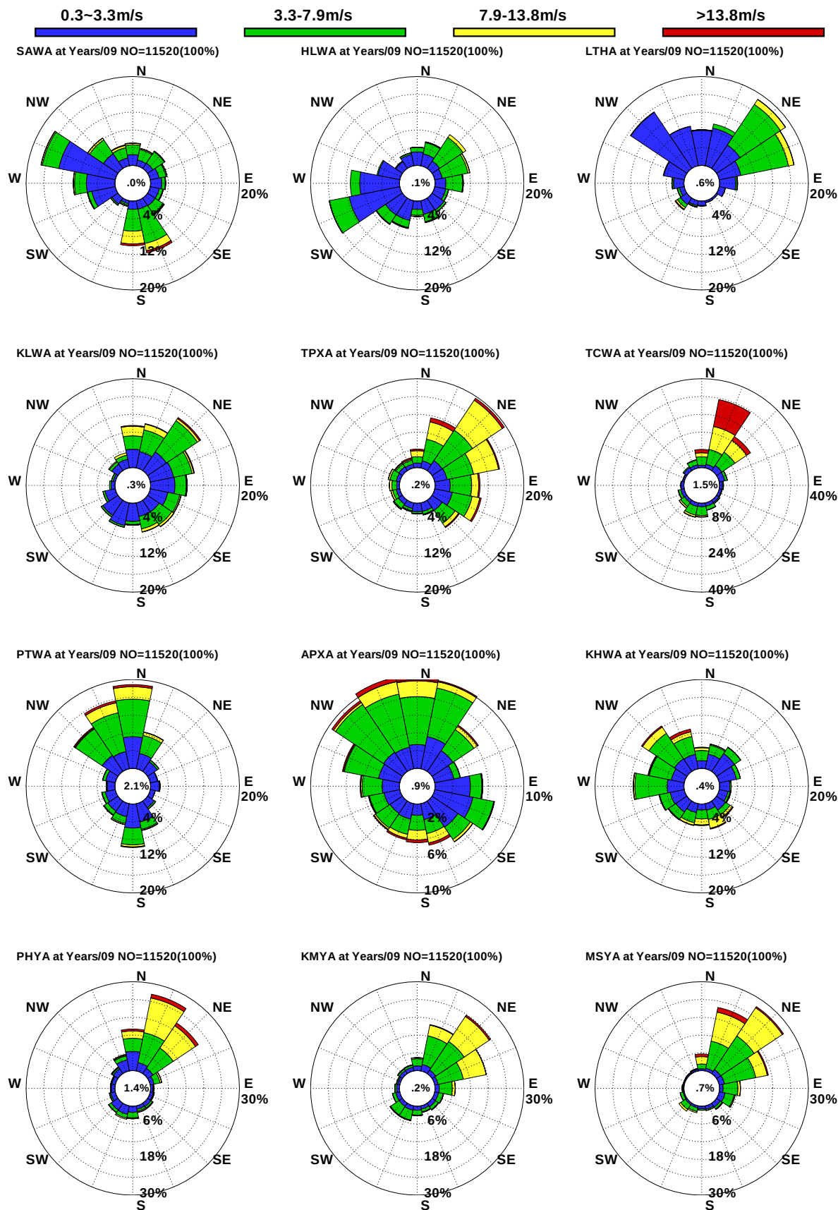
圖10.20 12港域歷年 9 月觀測風玫瑰比較圖
