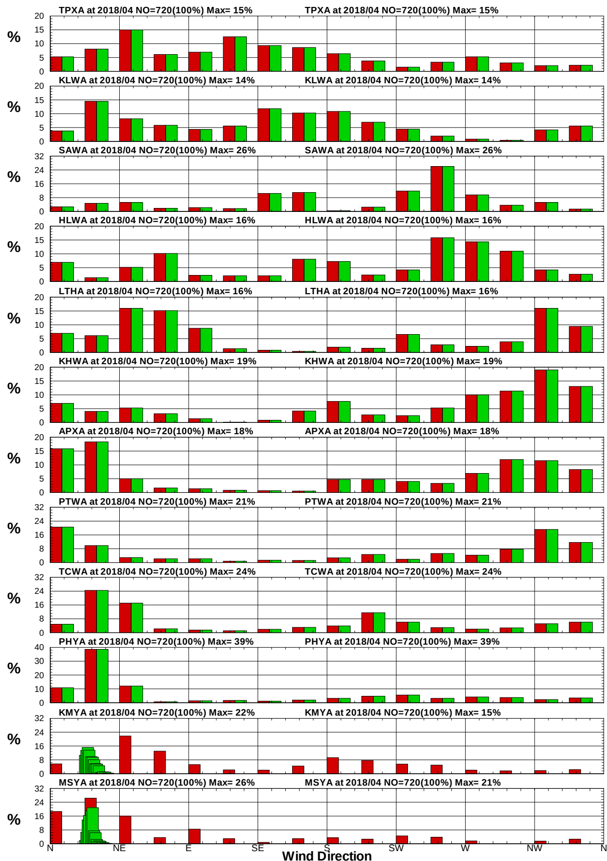
圖9.10 12港域2018年4月年12月風向統計方塊圖
