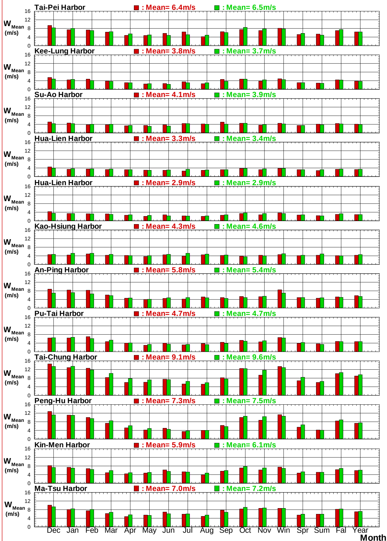
圖8.3a 2018及歷年12港域主要測站每月(季)平均風速比較圖
