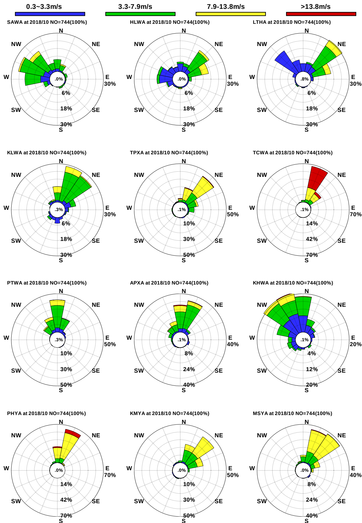
圖10.21 12港域2018年10月觀測風玫瑰比較圖
