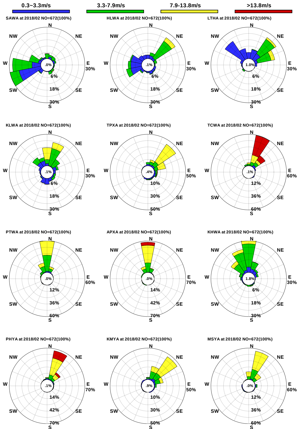
圖10.5 12港域2018年2月觀測風玫瑰比較圖
