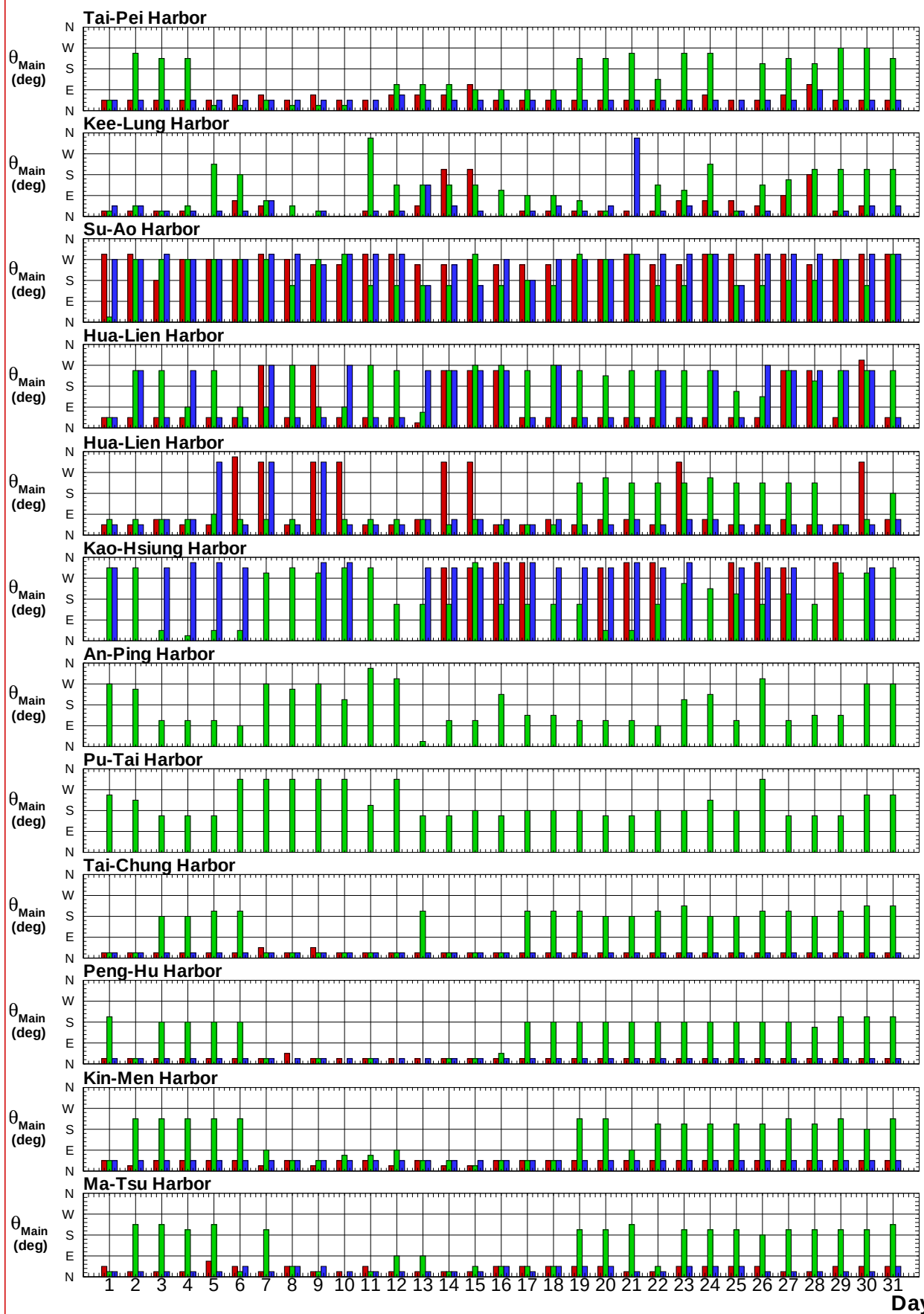
圖8.6e 2018年12港域冬, 夏及整年主要測站每日主要風向比較圖
