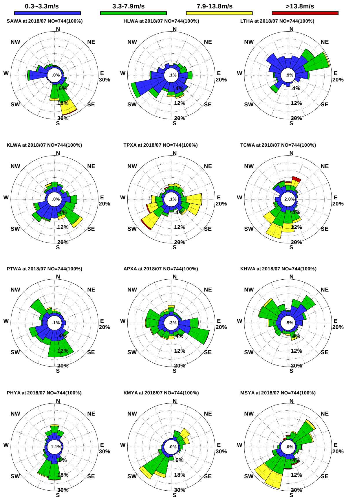
圖10.15 12港域2018年7月觀測風玫瑰比較圖
