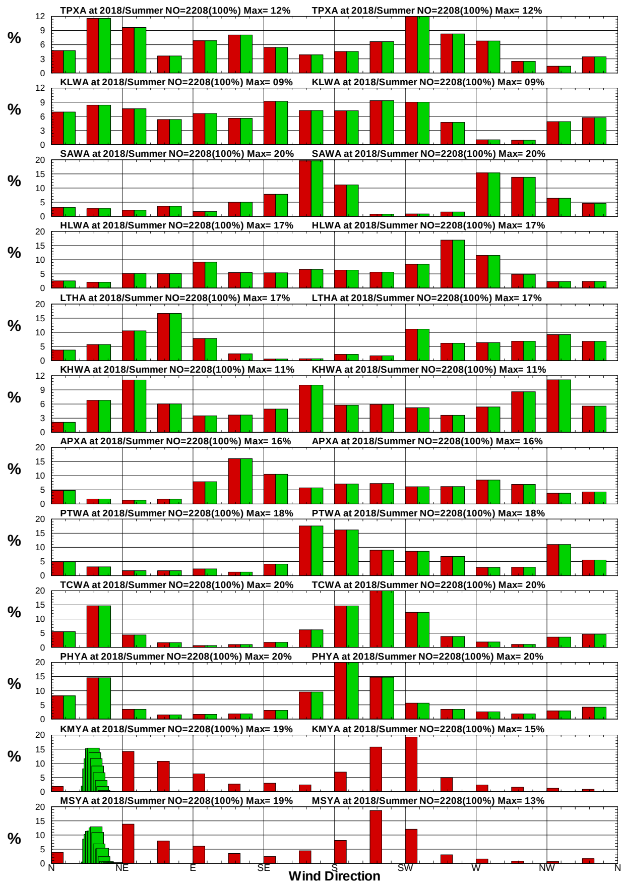
圖9.30 12港域2018年夏季年12月風向統計方塊圖
