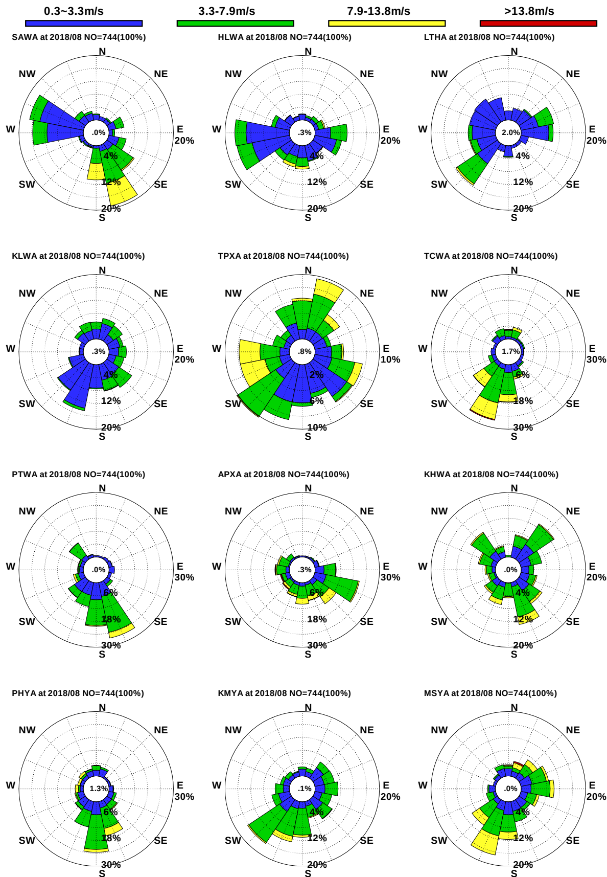
圖10.17 12港域2018年 8月觀測風玫瑰比較圖
