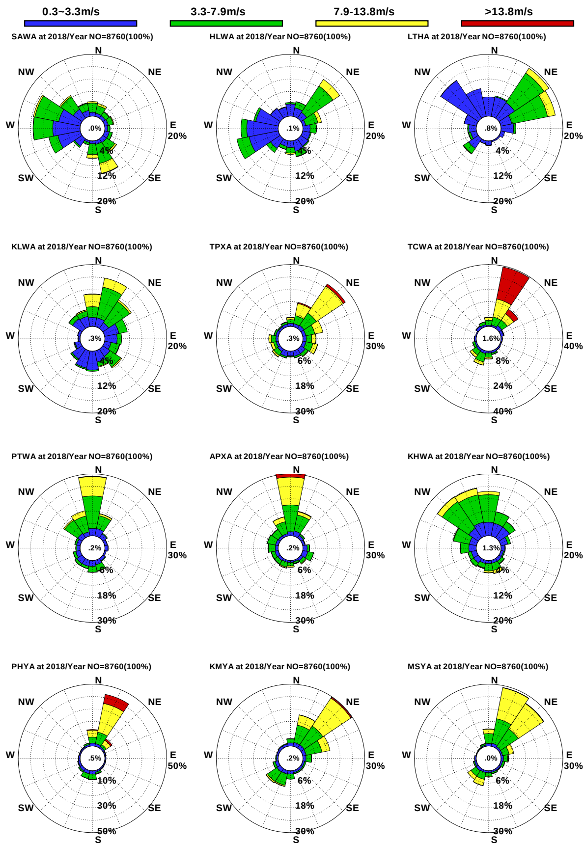
圖10.33 12港域2018年整年觀測風玫瑰比較圖
