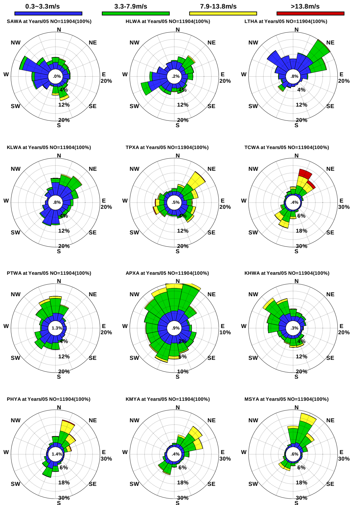
圖10.12 12港域歷年 5月觀測風玫瑰比較圖
