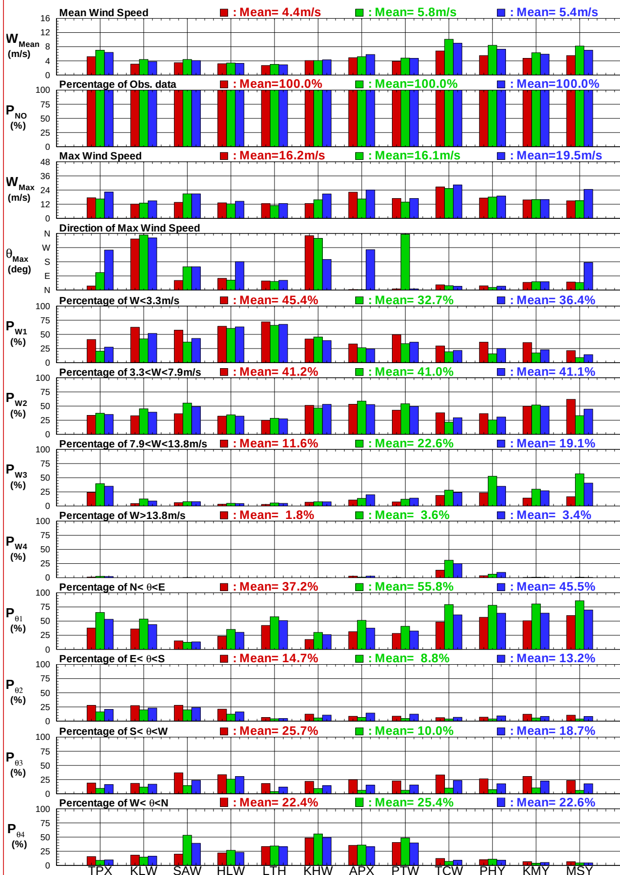
圖8.2c 12個港域2018年主要測站春、秋及整年風速 (向) 比較圖
