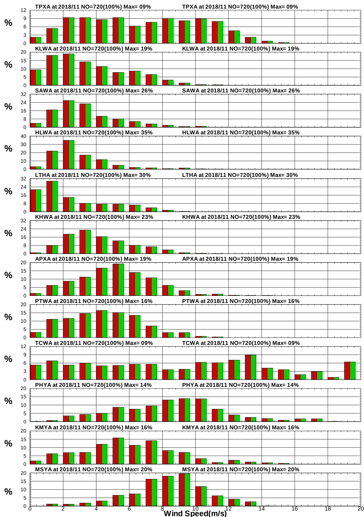
圖9.23 12港域2018年11月12月風速統計方塊圖
