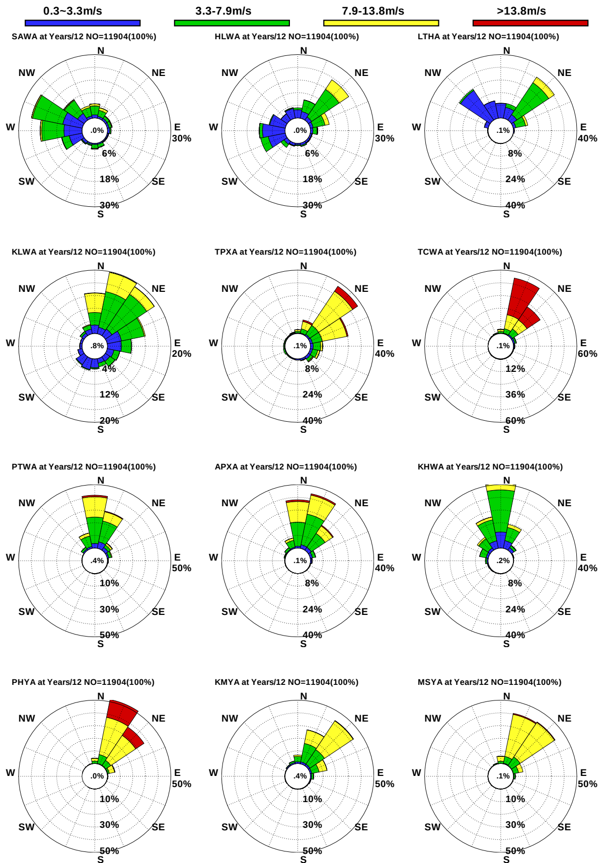
圖10.2 12港域歷年12月觀測風玫瑰比較圖
