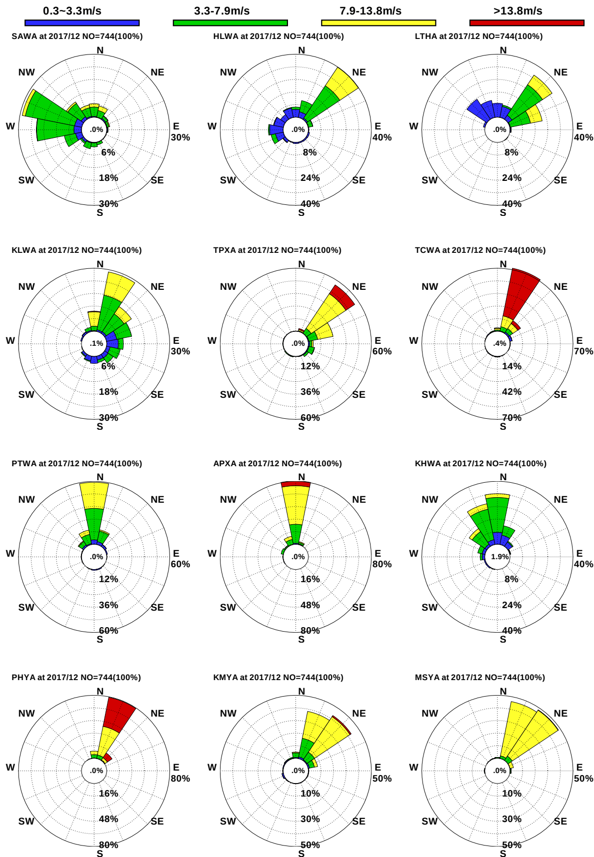
圖10.1 12港域2017年12月觀測風玫瑰比較圖
