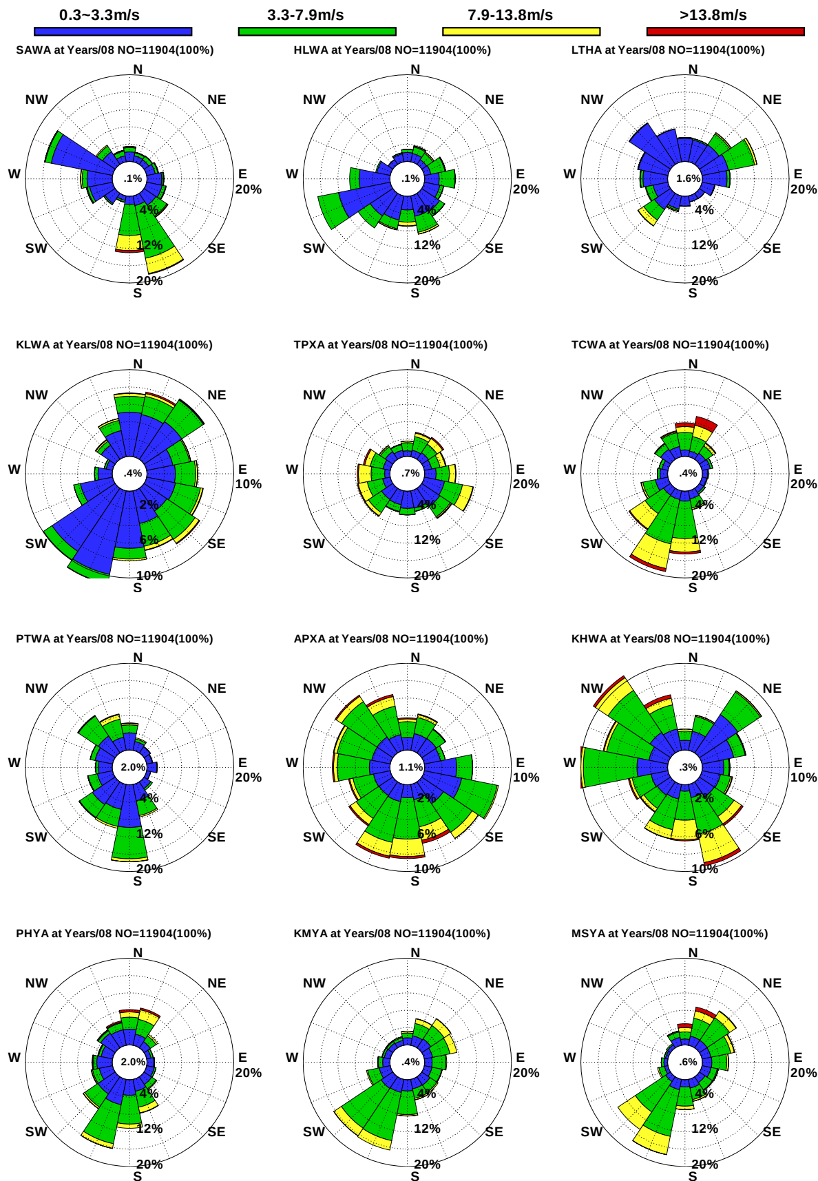
圖10.18 12港域歷年 8 月觀測風玫瑰比較圖
