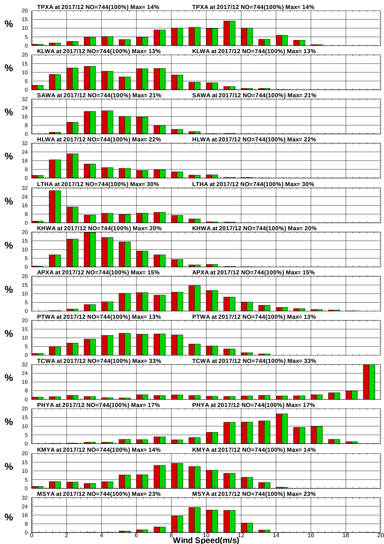
圖9.1 12港域2017年12月風速統計方塊圖
