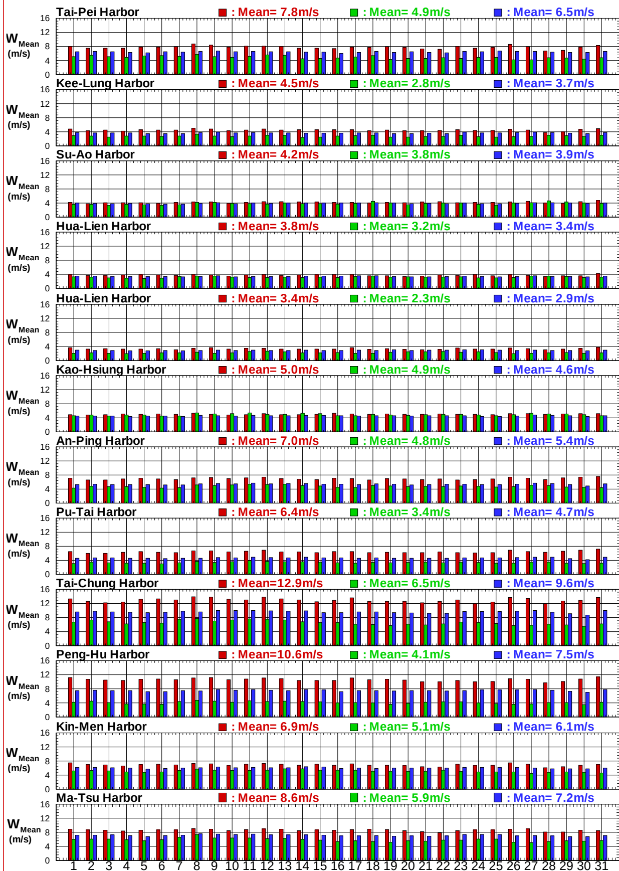
圖8.7a 歷年12港域冬, 夏及整年主要測站每日平均風速比較圖
