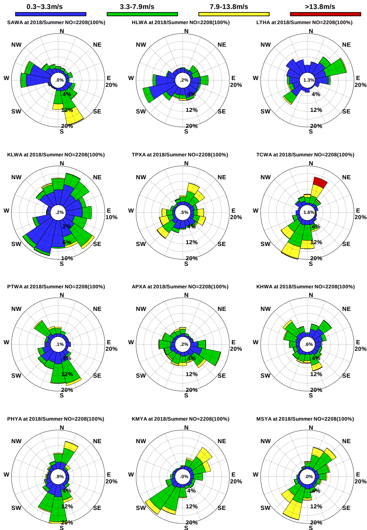
圖10.29 12港域2018年夏季觀測風玫瑰比較圖
