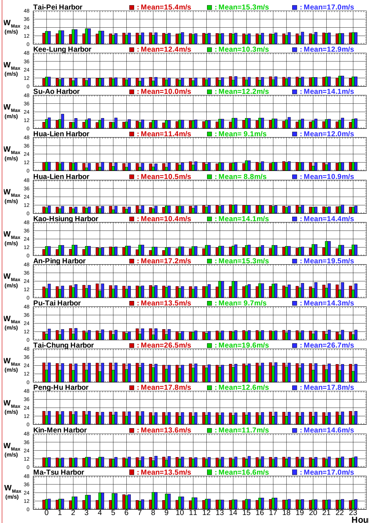
圖8.4c 2018年12港域冬、夏及整年主要測站逐時最大風速比較圖
