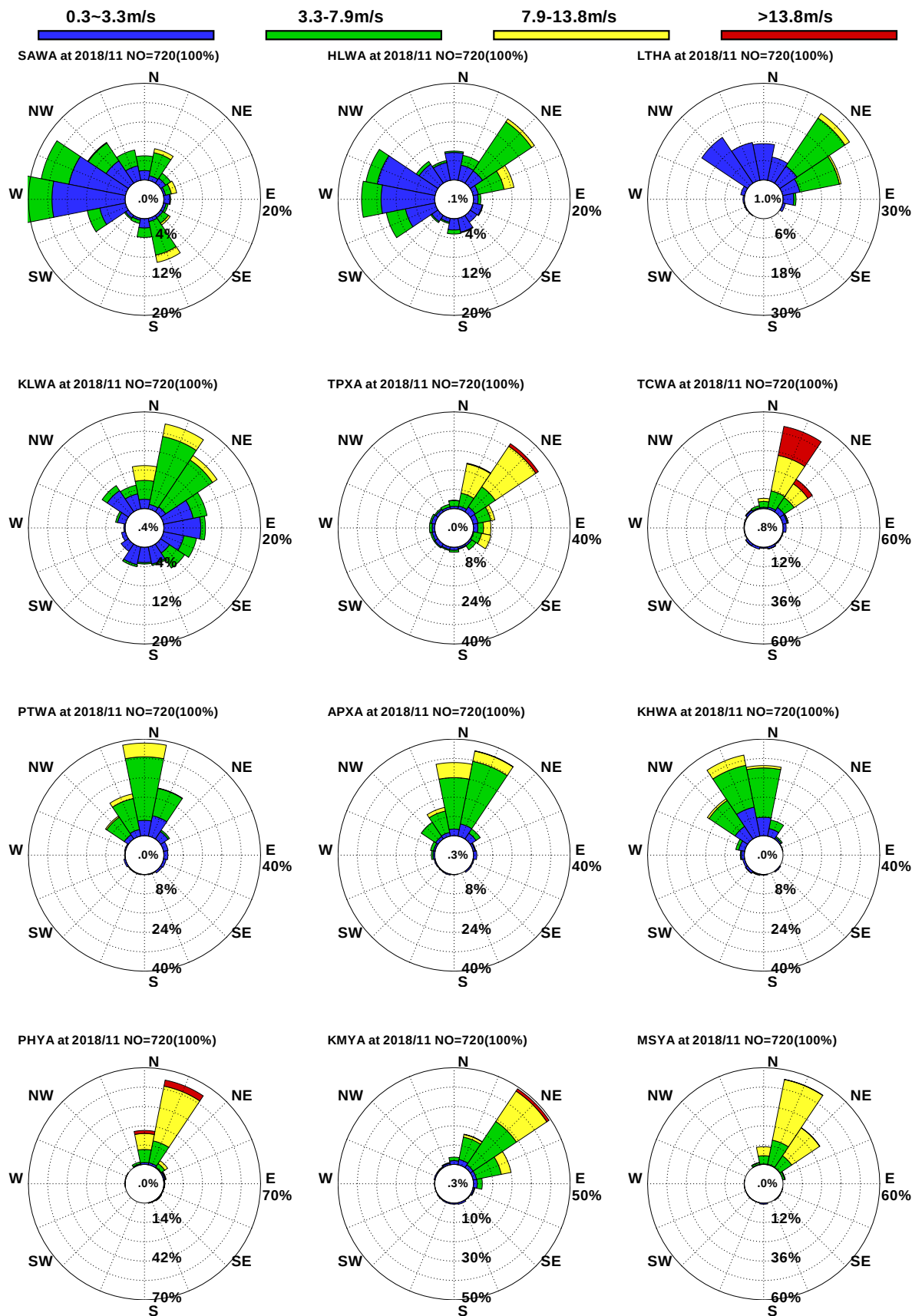
圖10.23 12港域2018年11月觀測風玫瑰比較圖
