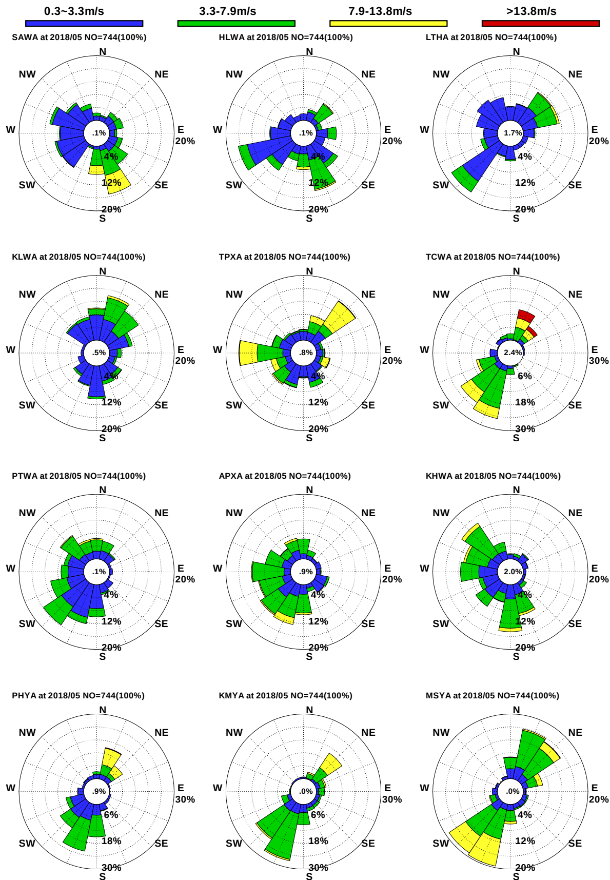
圖10.11 12港域2018年 5月觀測風玫瑰比較圖
