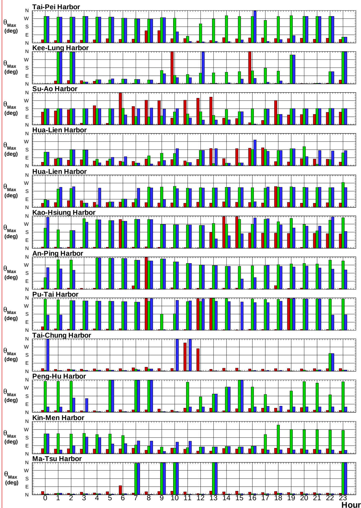
圖8.5d 歷年12港域冬, 夏及整年主要測站逐時最大風速之風向圖
