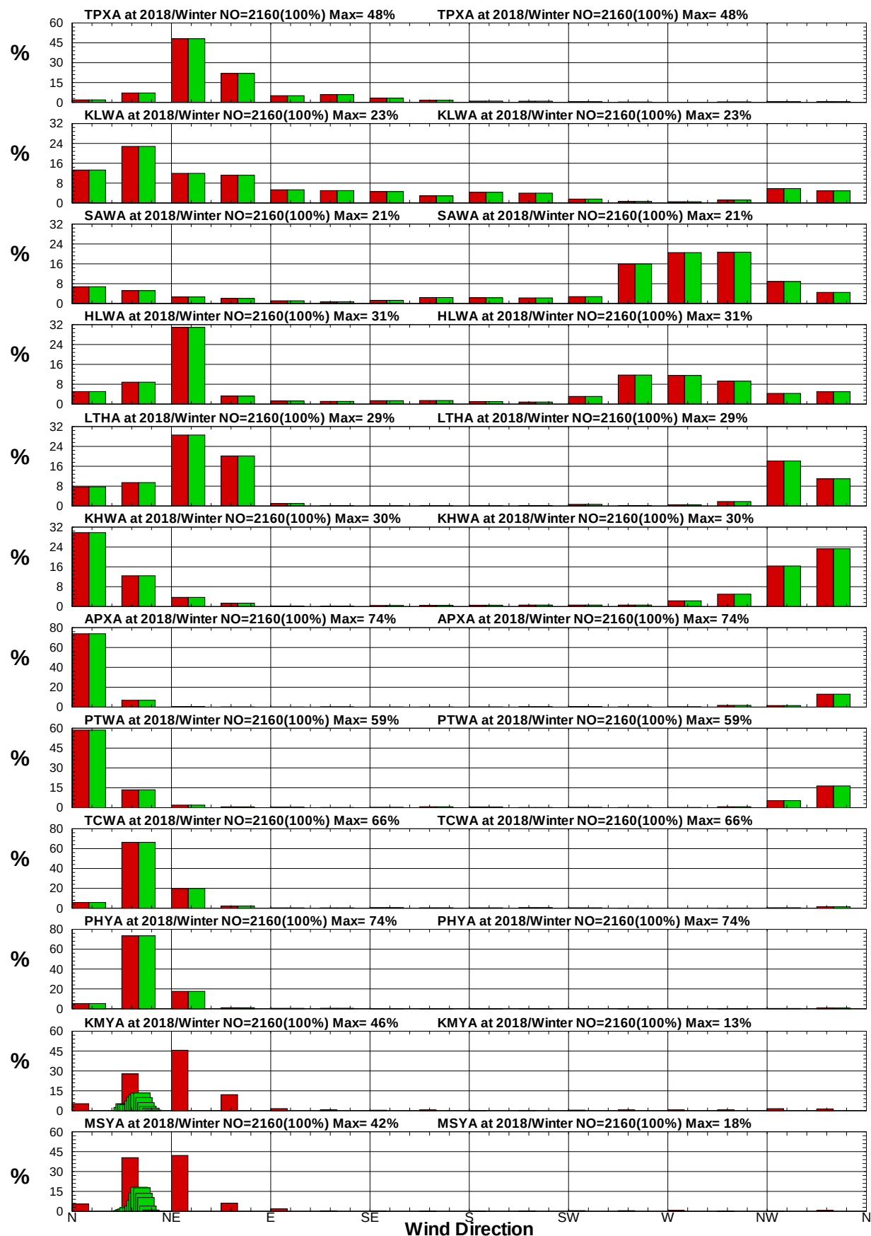
圖9.26 12港域2018年冬季年12月風向統計方塊圖
