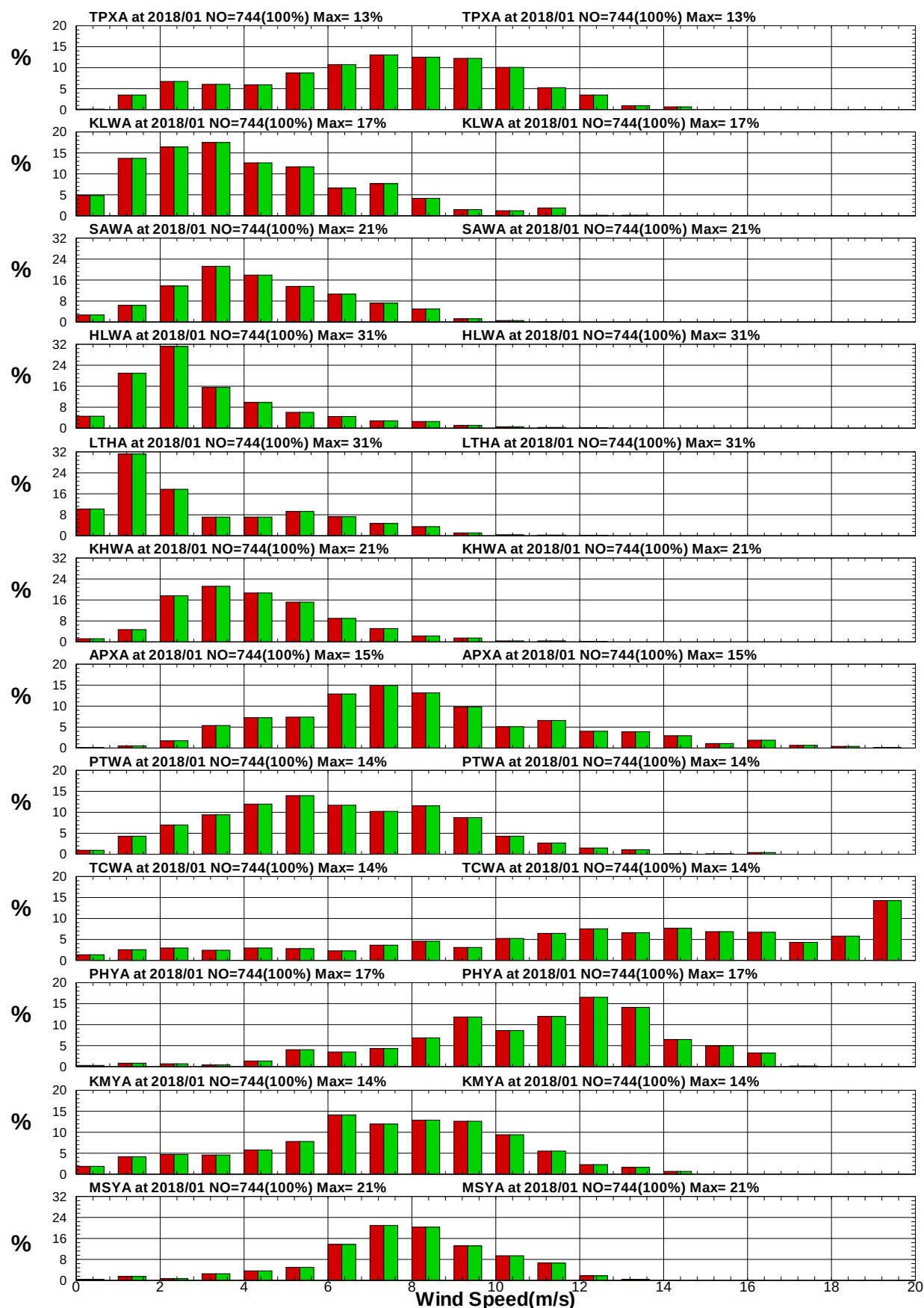
圖9.3 12港域2018年 1月年12月風速統計方塊圖
