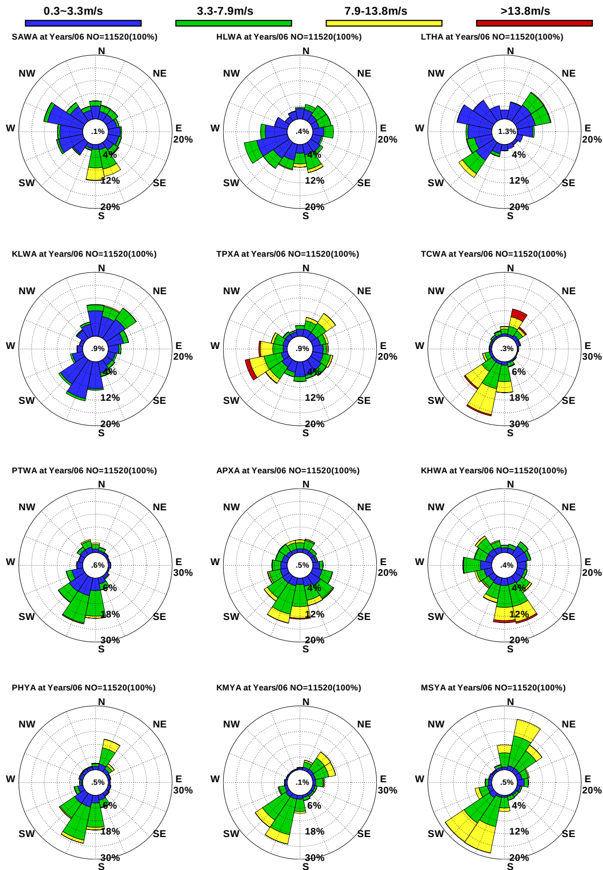
圖10.14 12港域歷年 6 月觀測風玫瑰比較圖
