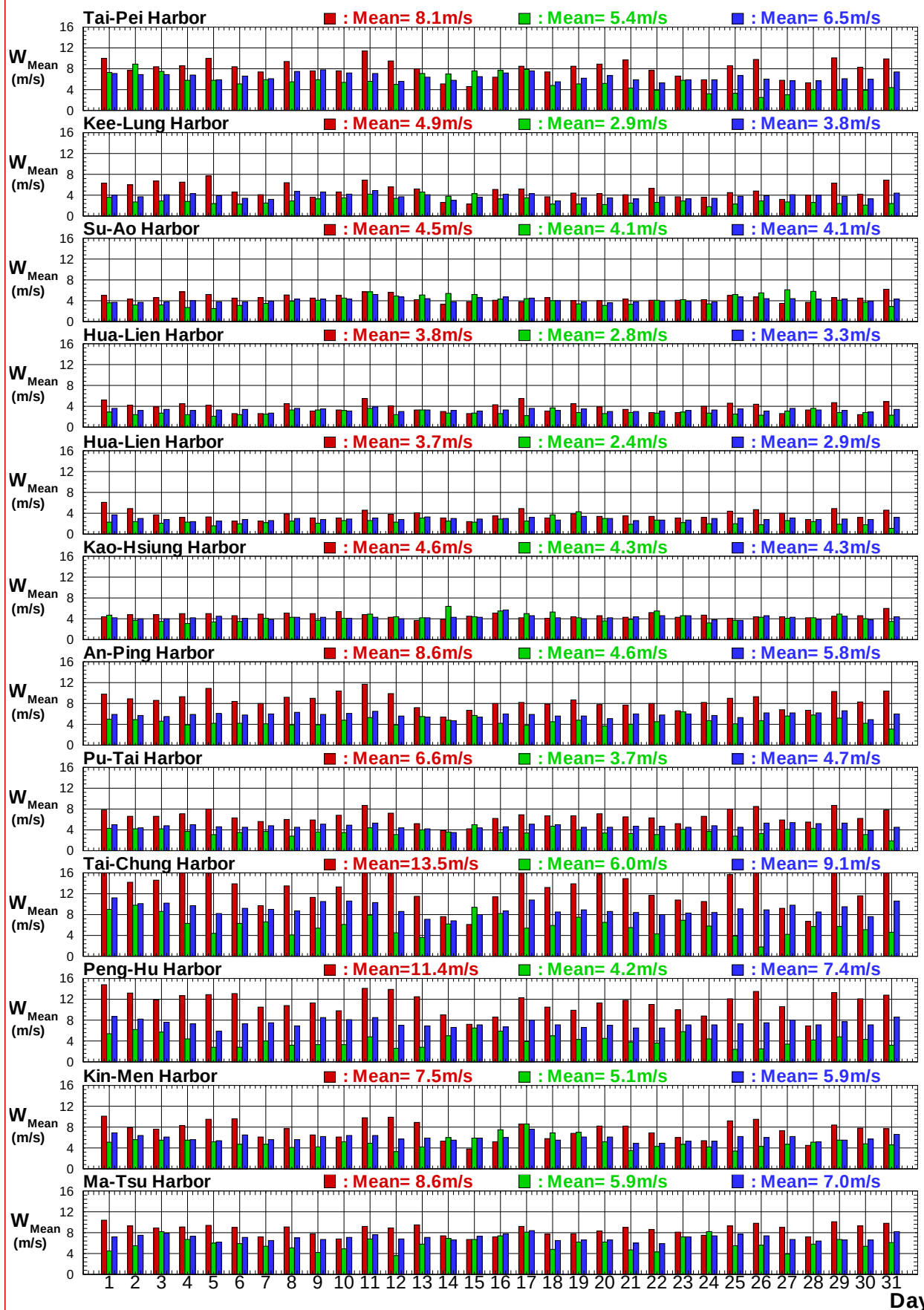
圖8.6a 2018年12港域冬, 夏及整年主要測站每日平均風速比較圖
