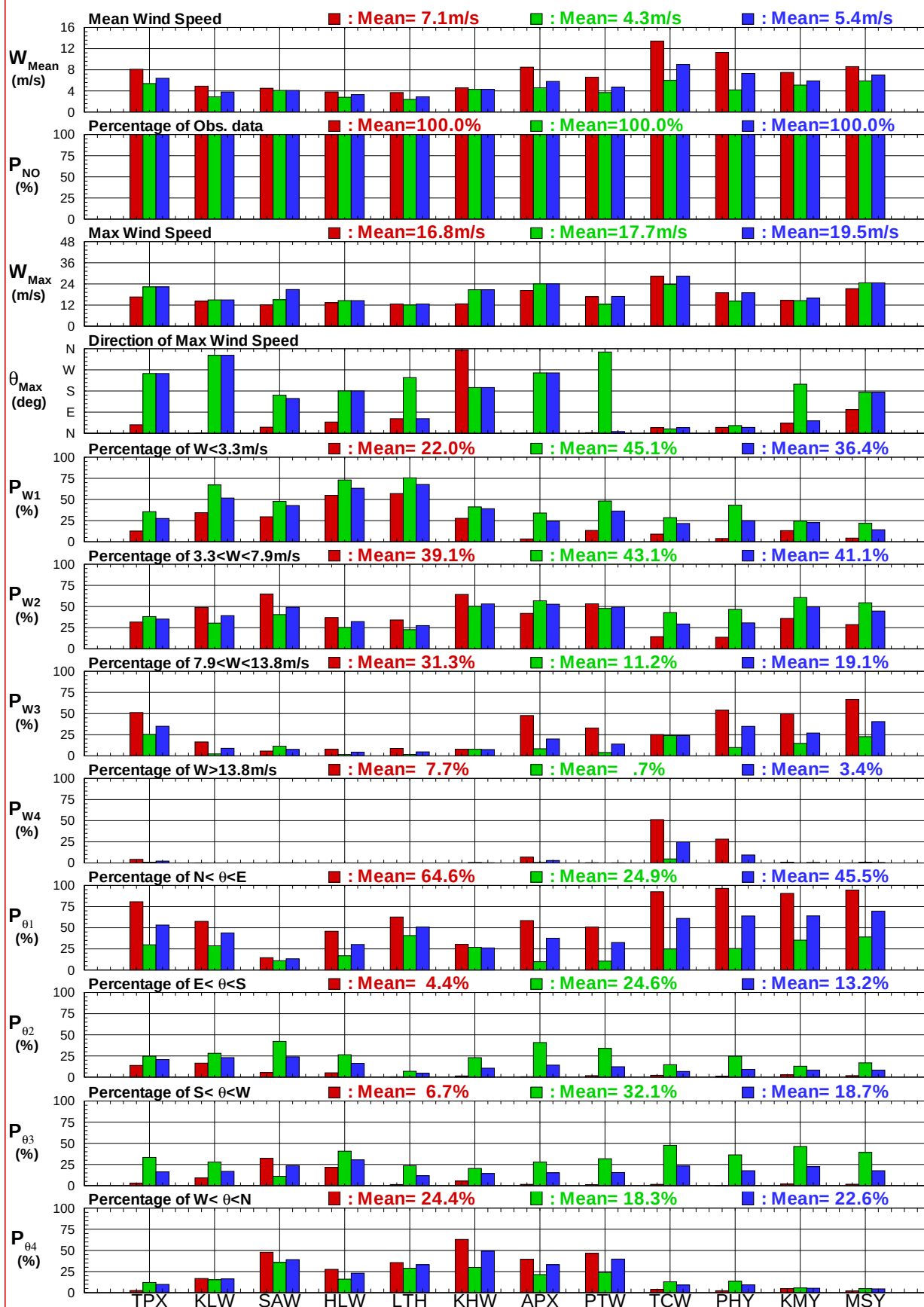
圖8.2a 12個港域2018年主要測站冬、夏及整年風速 (向) 比較圖
