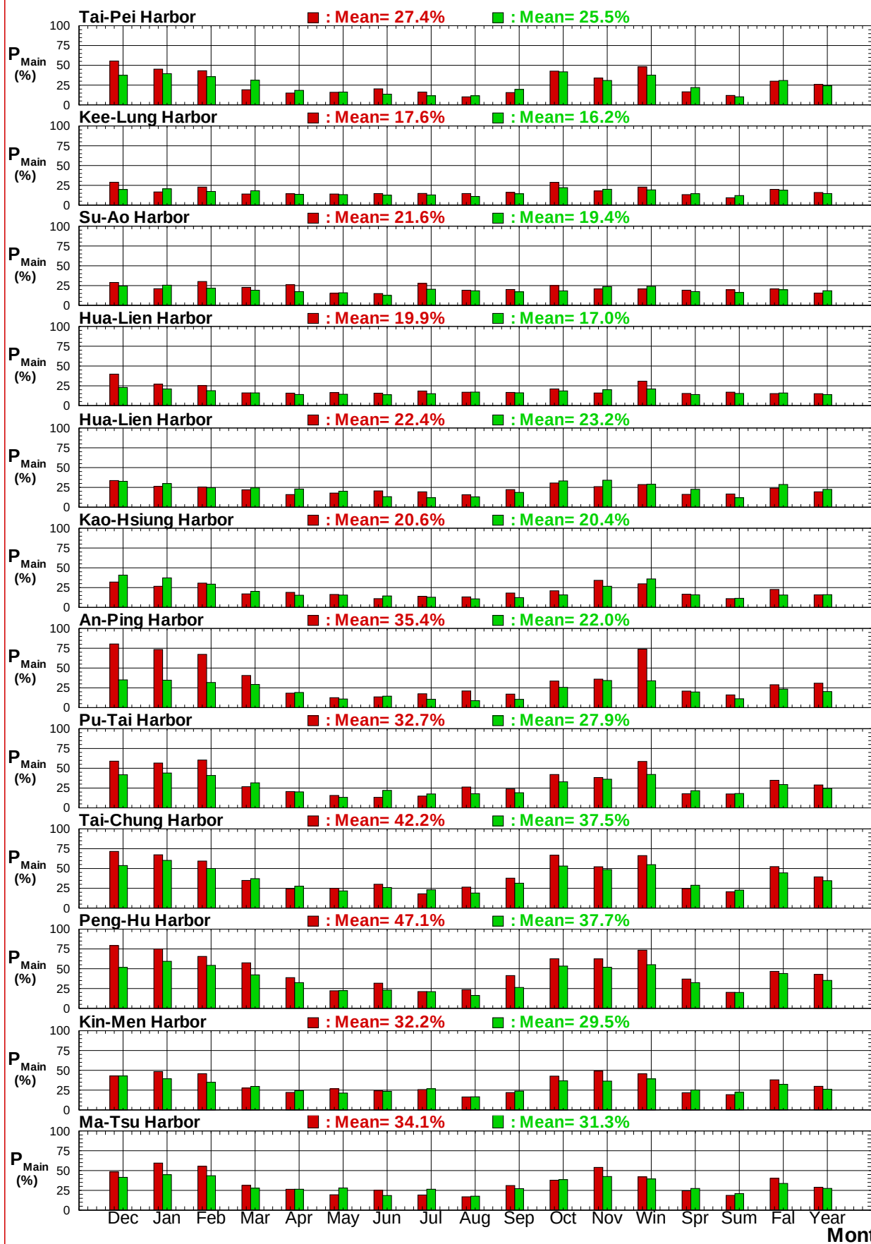
圖8.3f 2018及歷年12港域主要測站每月(季)主要風向百分比圖
