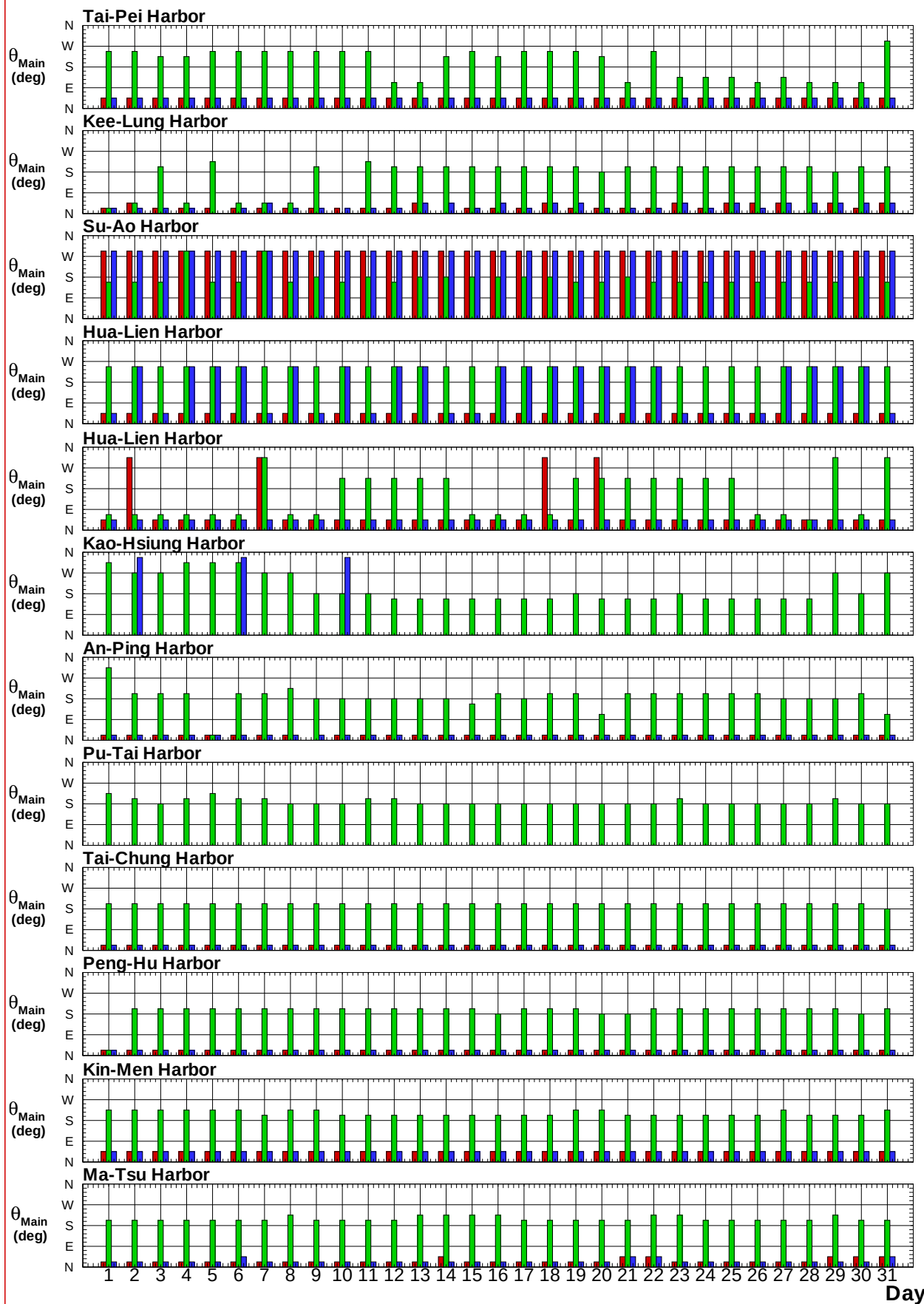
圖8.7e 歷年12港域冬, 夏及整年主要測站每日主要風向比較圖
