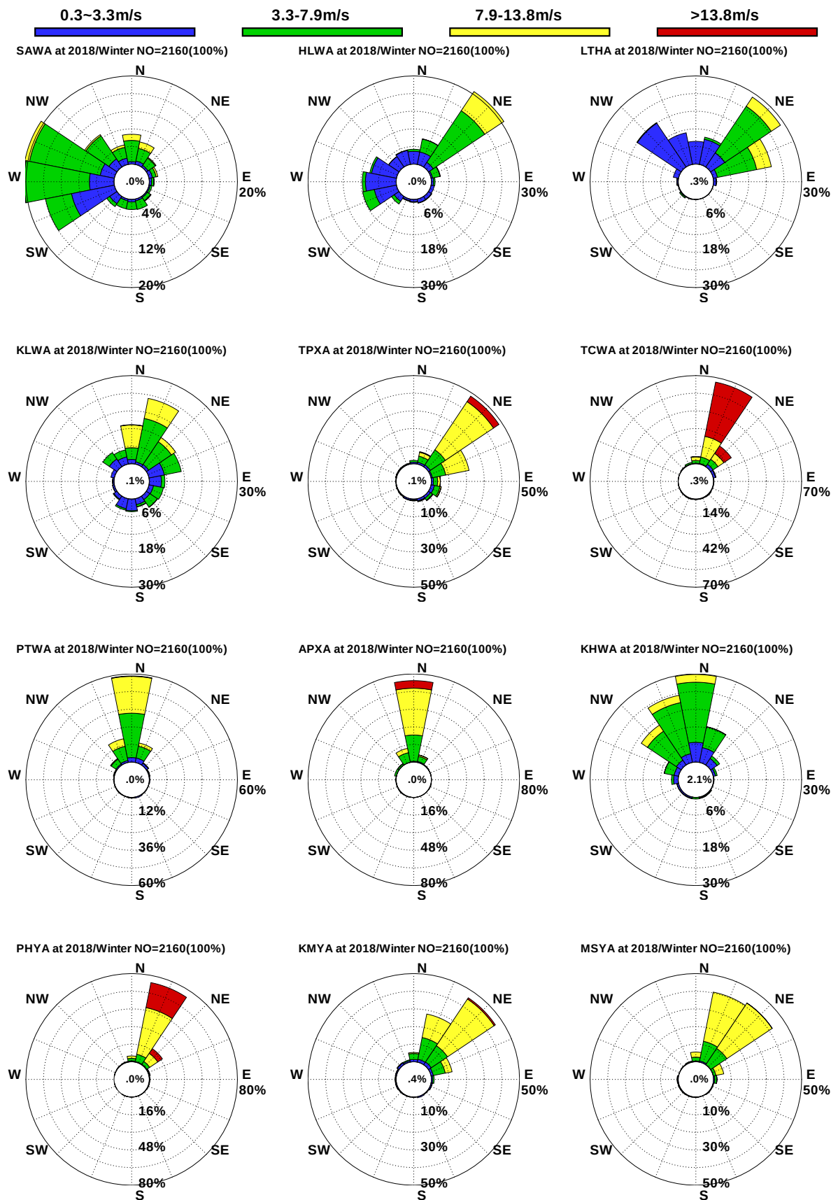
圖10.25 12港域2018年冬季觀測風玫瑰比較圖
