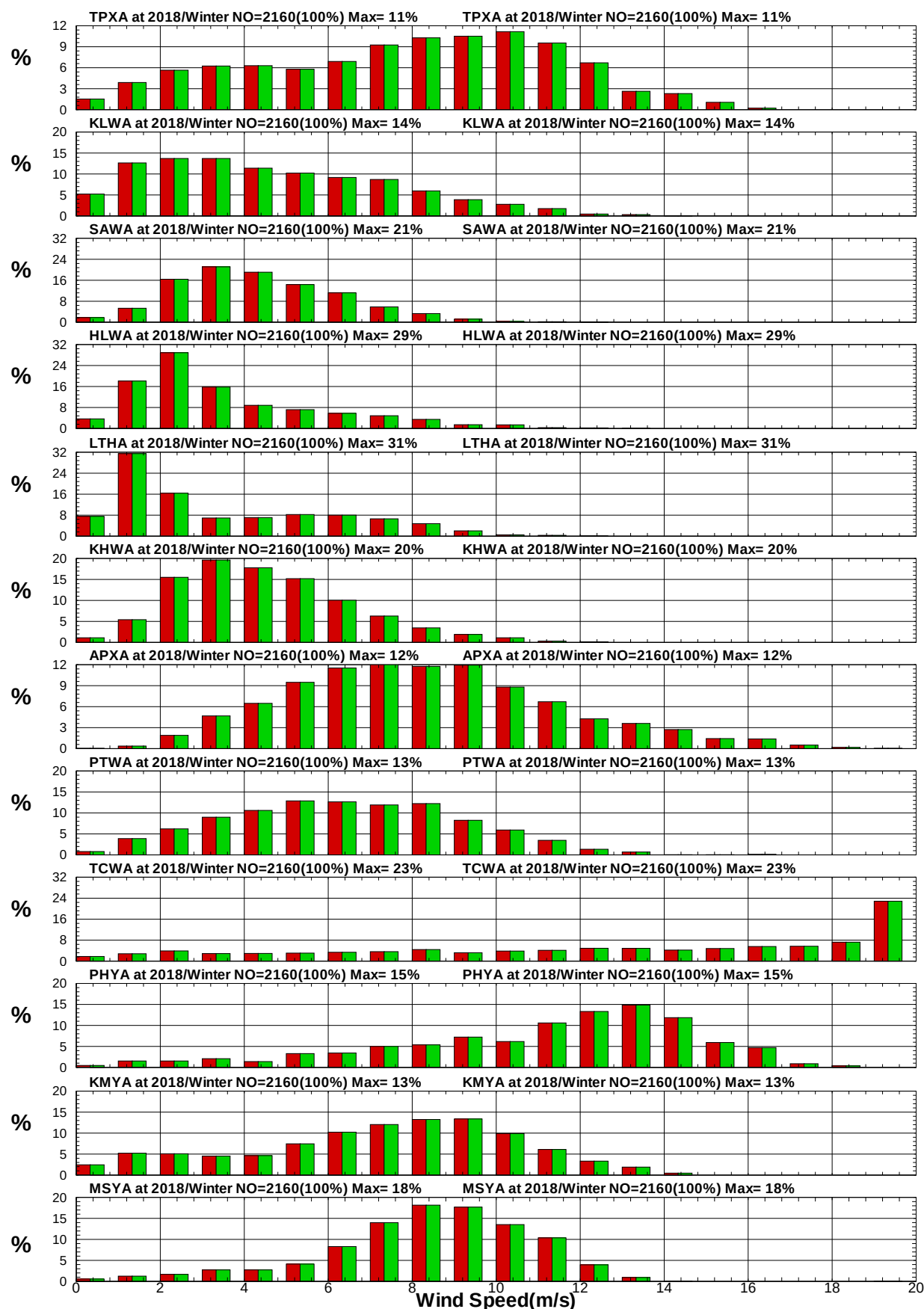
圖9.25 12港域2018年冬季年12月風速統計方塊圖
