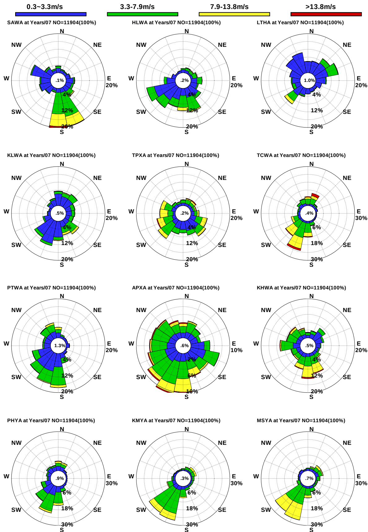
圖10.16 12港域歷年 7月觀測風玫瑰比較圖
