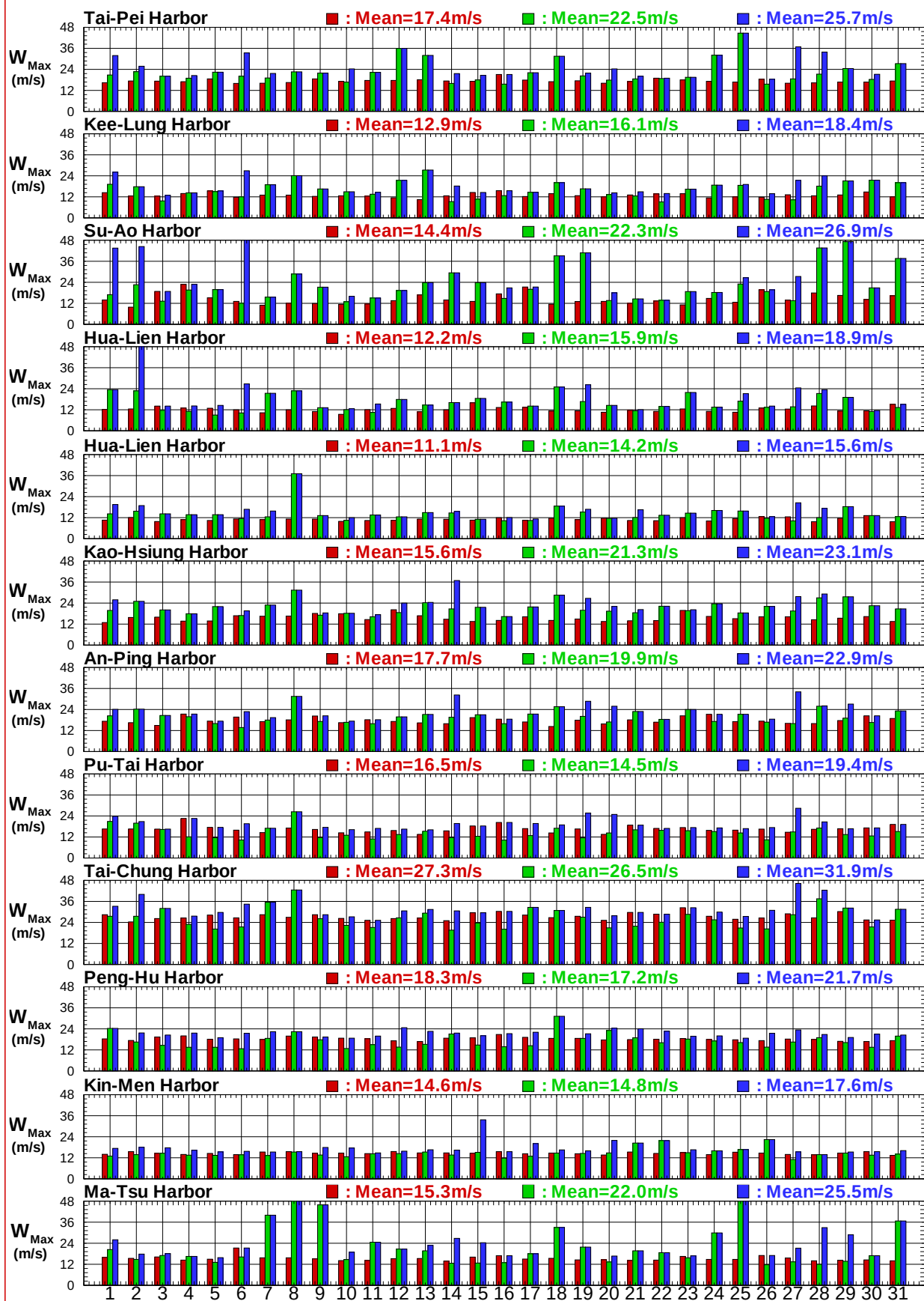
圖8.7c 歷年12港域冬, 夏及整年主要測站每日最大風速比較圖
