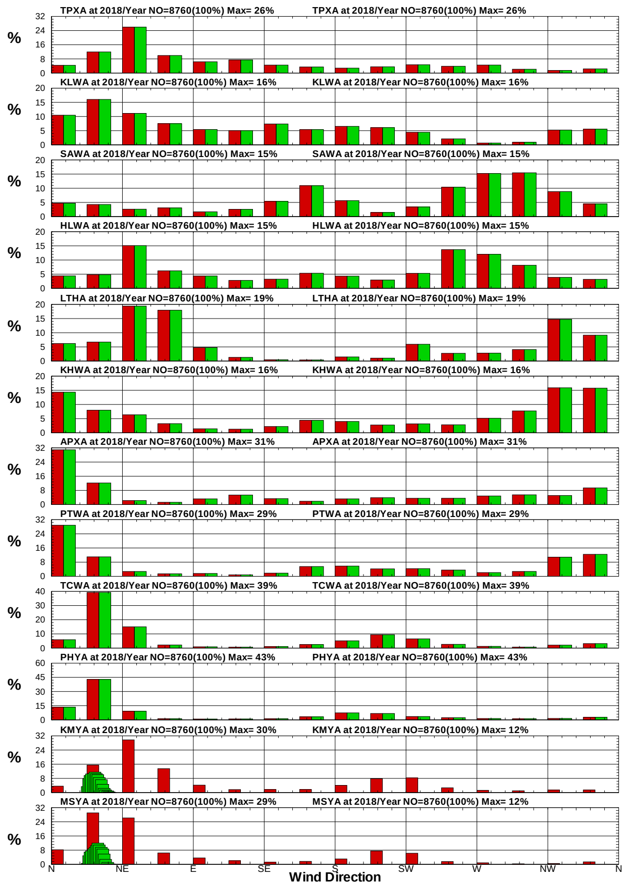
圖9.34 12港域2018年整年年12月風向統計方塊圖
