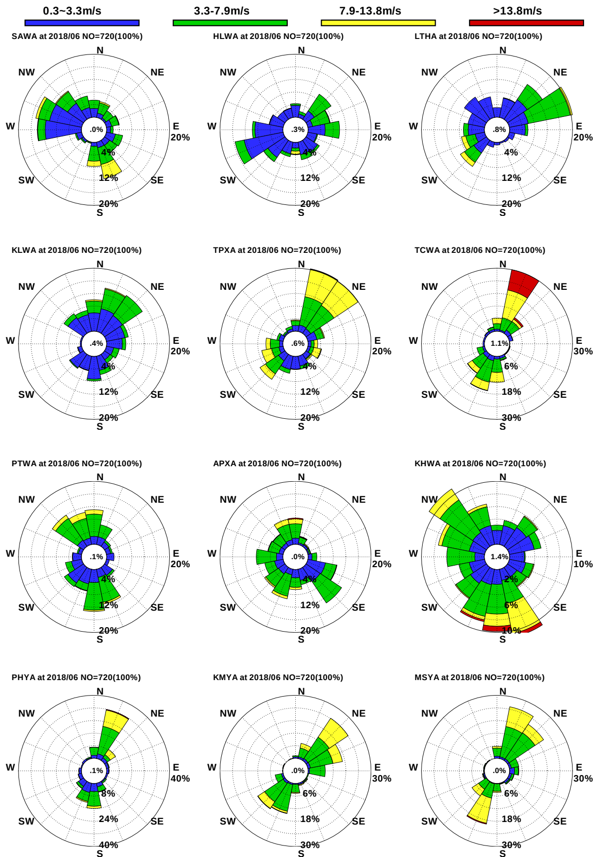
圖10.13 12港域2018年 6月觀測風玫瑰比較圖
