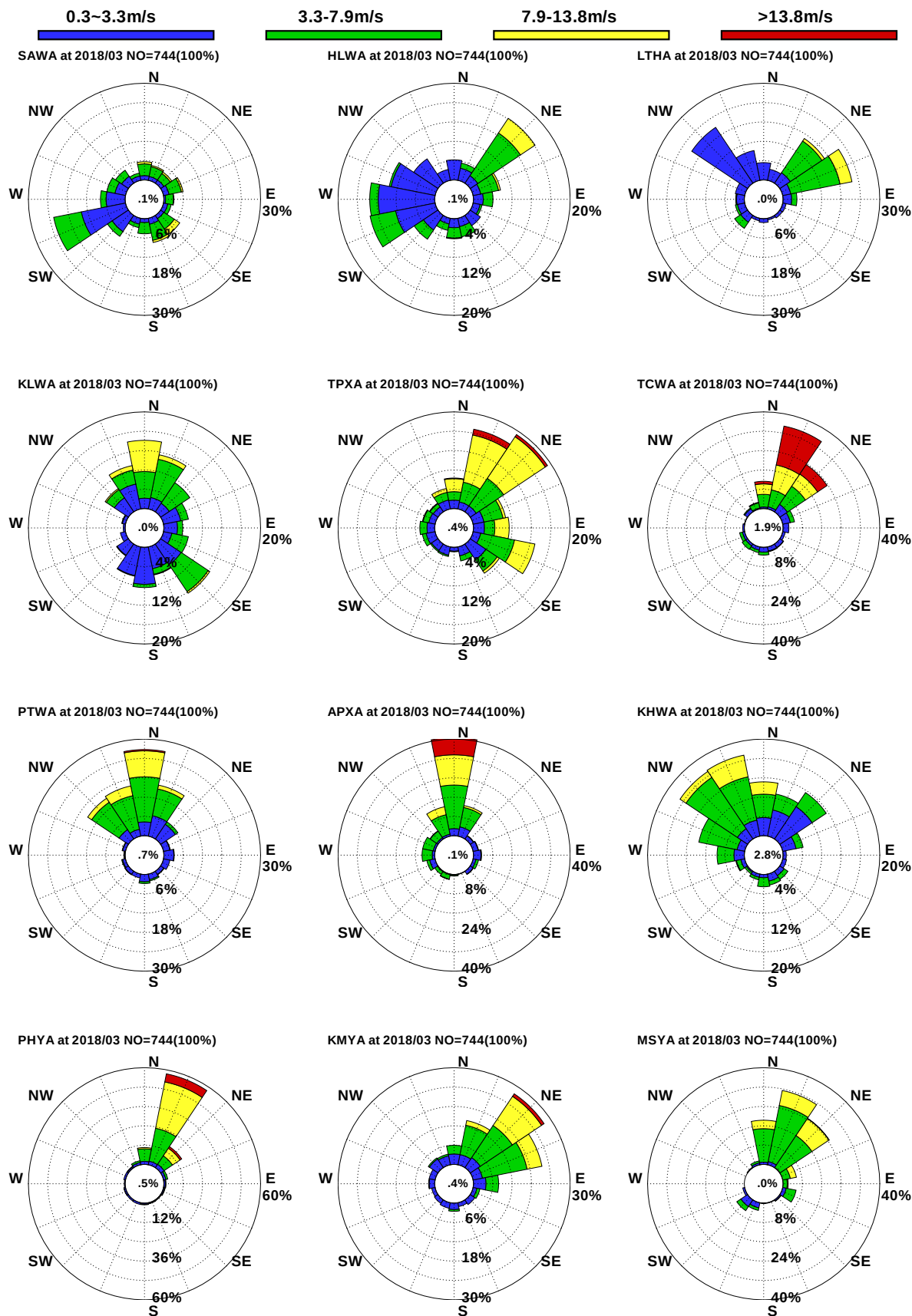
圖10.7 12港域2018年 3月觀測風玫瑰比較圖
