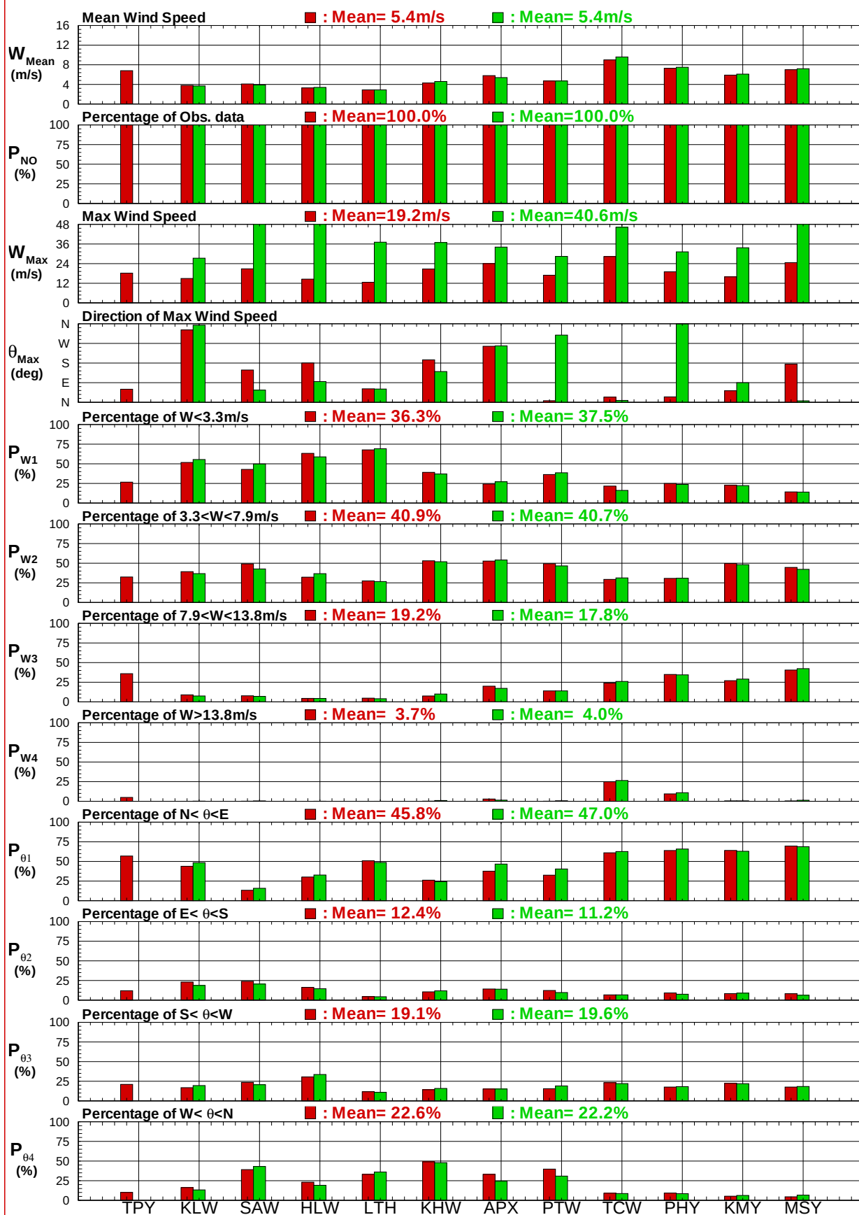
圖8.1e 12個港域2018及歷年主要測站整年風速(向)比較圖
