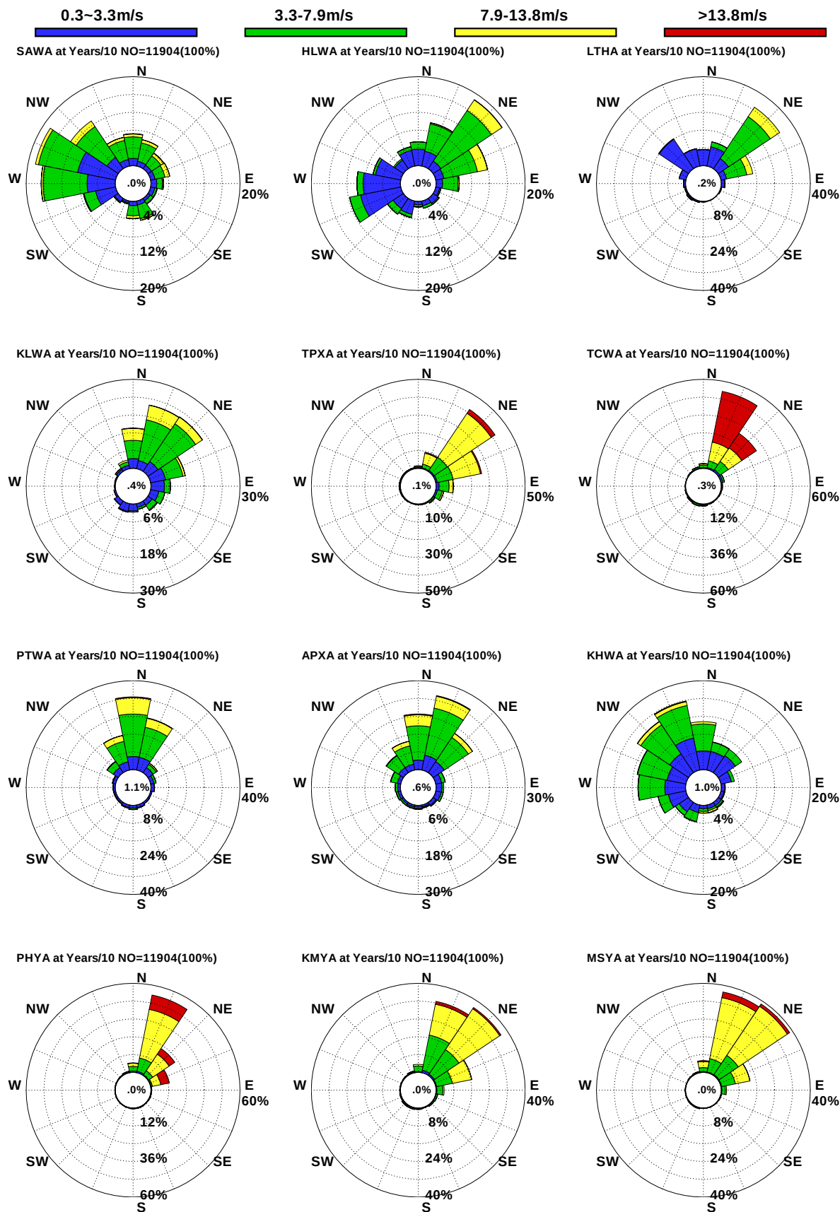
圖10.22 12港域歷年10月觀測風玫瑰比較圖
