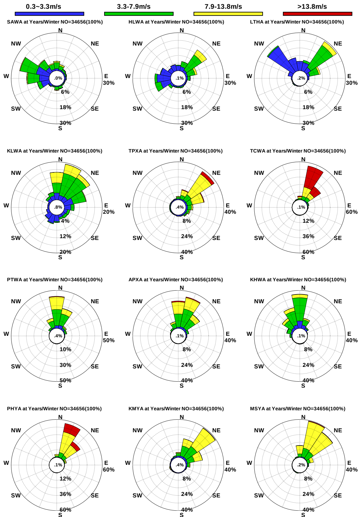
圖10.26 12港域歷年冬季觀測風玫瑰比較圖
