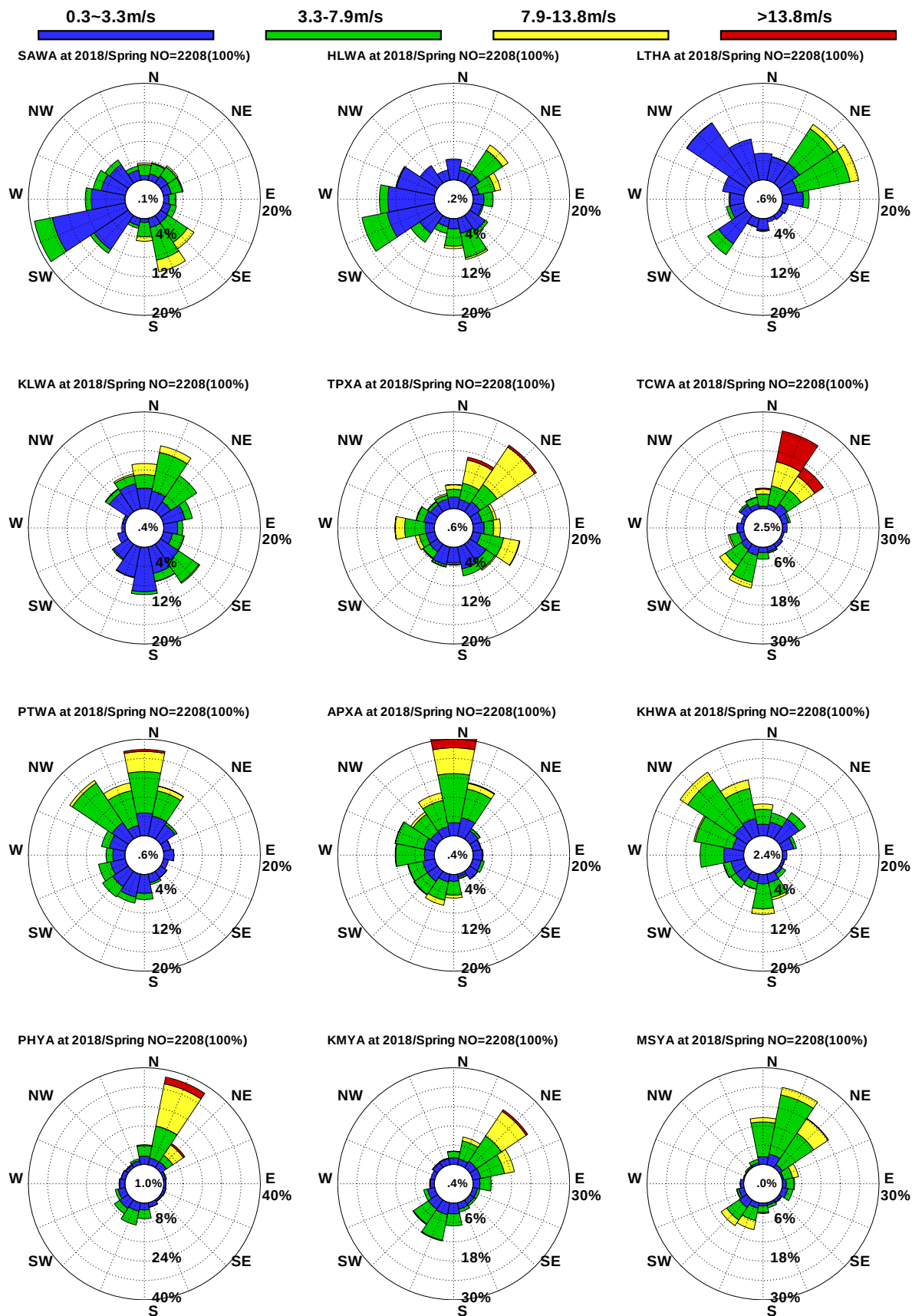
圖10.27 12港域2018年春季觀測風玫瑰比較圖
