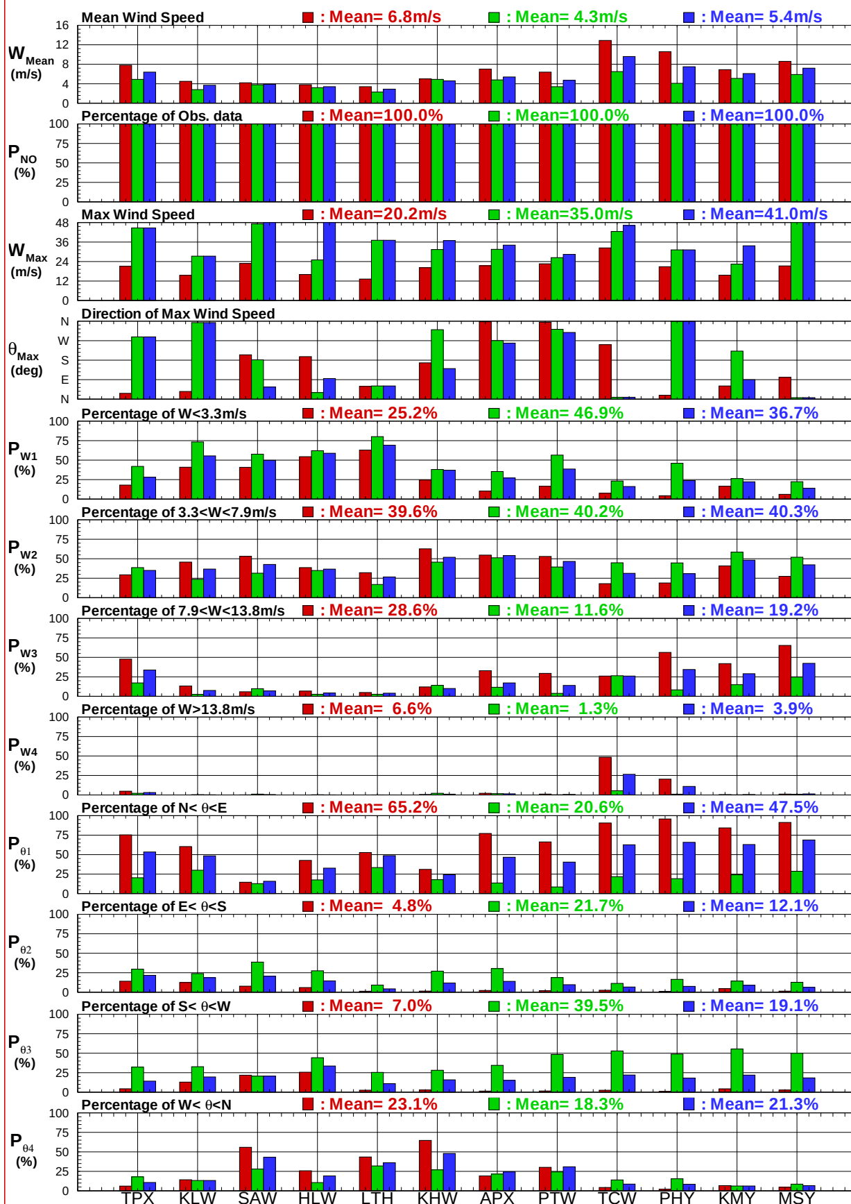
圖8.2b 12個港域歷年主要測站冬, 夏及整年風速 (向) 比較圖
