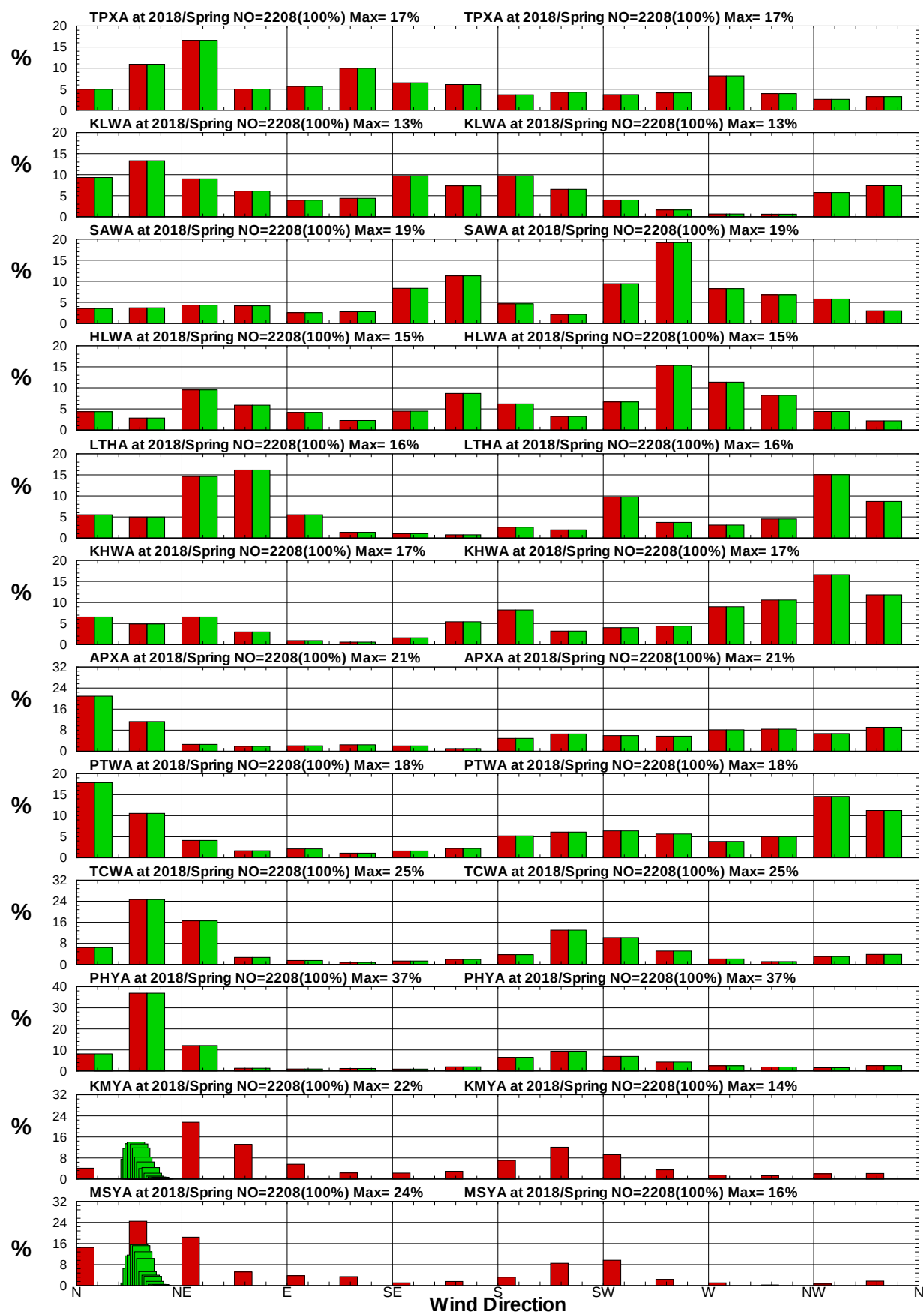
圖9.28 12港域2018年春季年12月風向統計方塊圖
