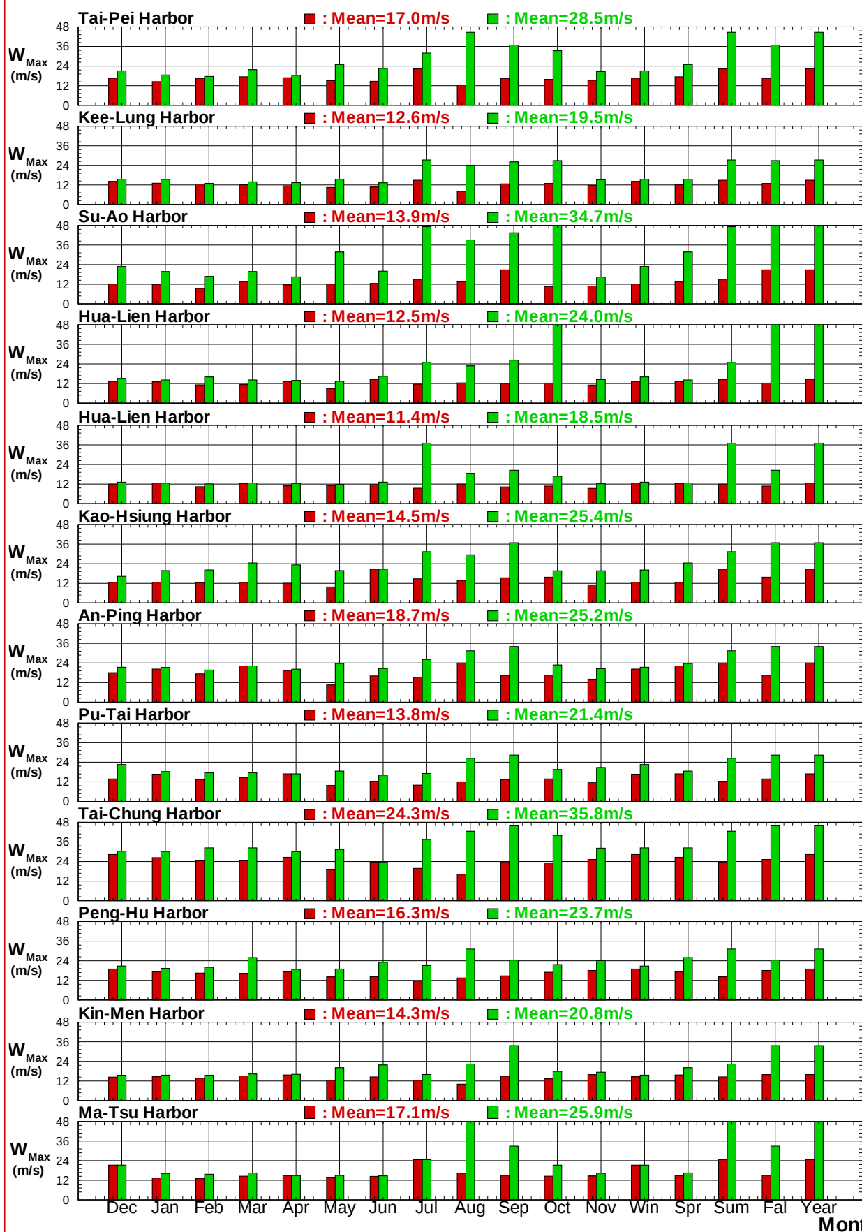
圖8.3c 2018及歷年12港域主要測站每月(季)最大風速比較圖
