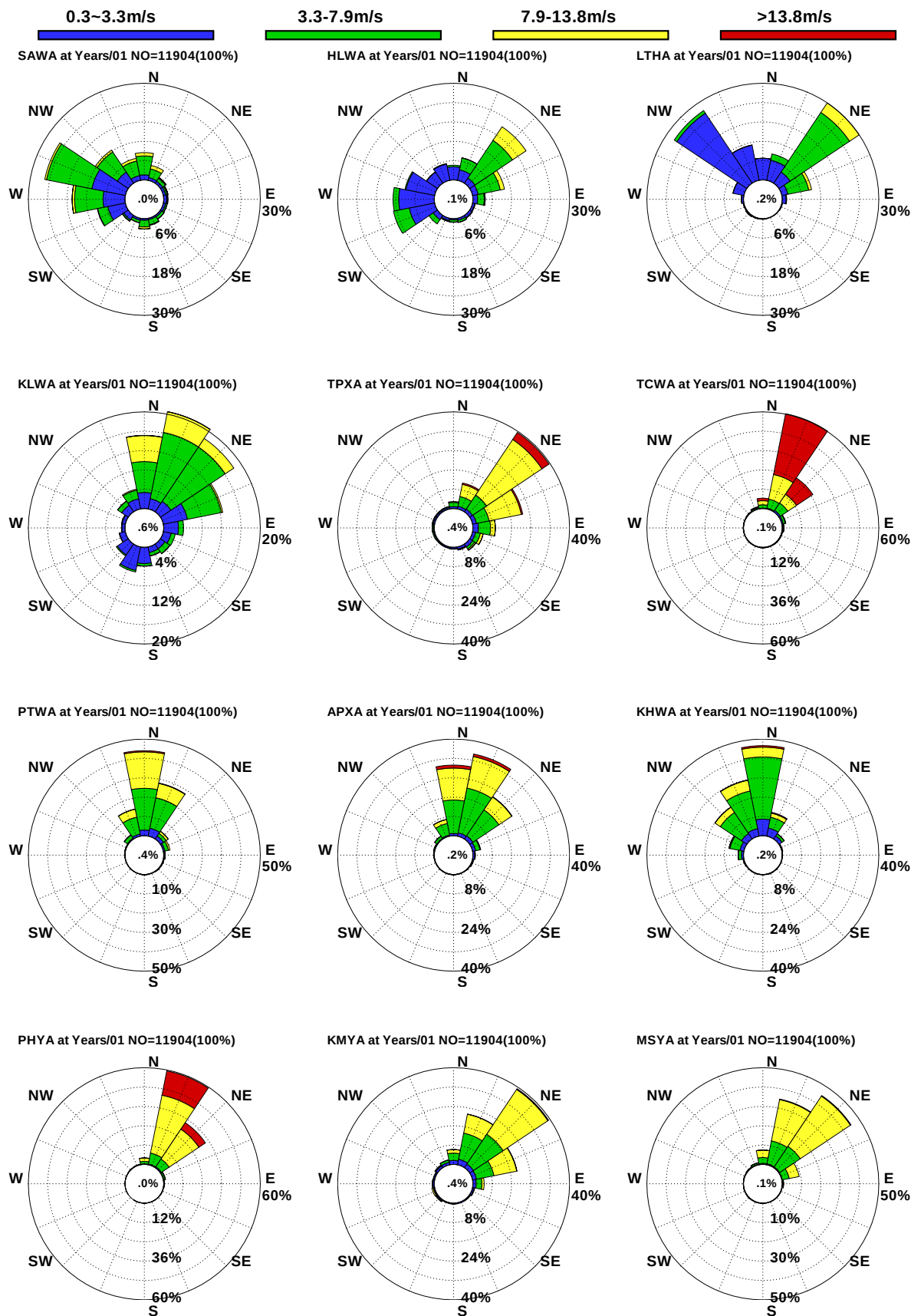
圖10.4 12港域歷年 1 月觀測風玫瑰比較圖
