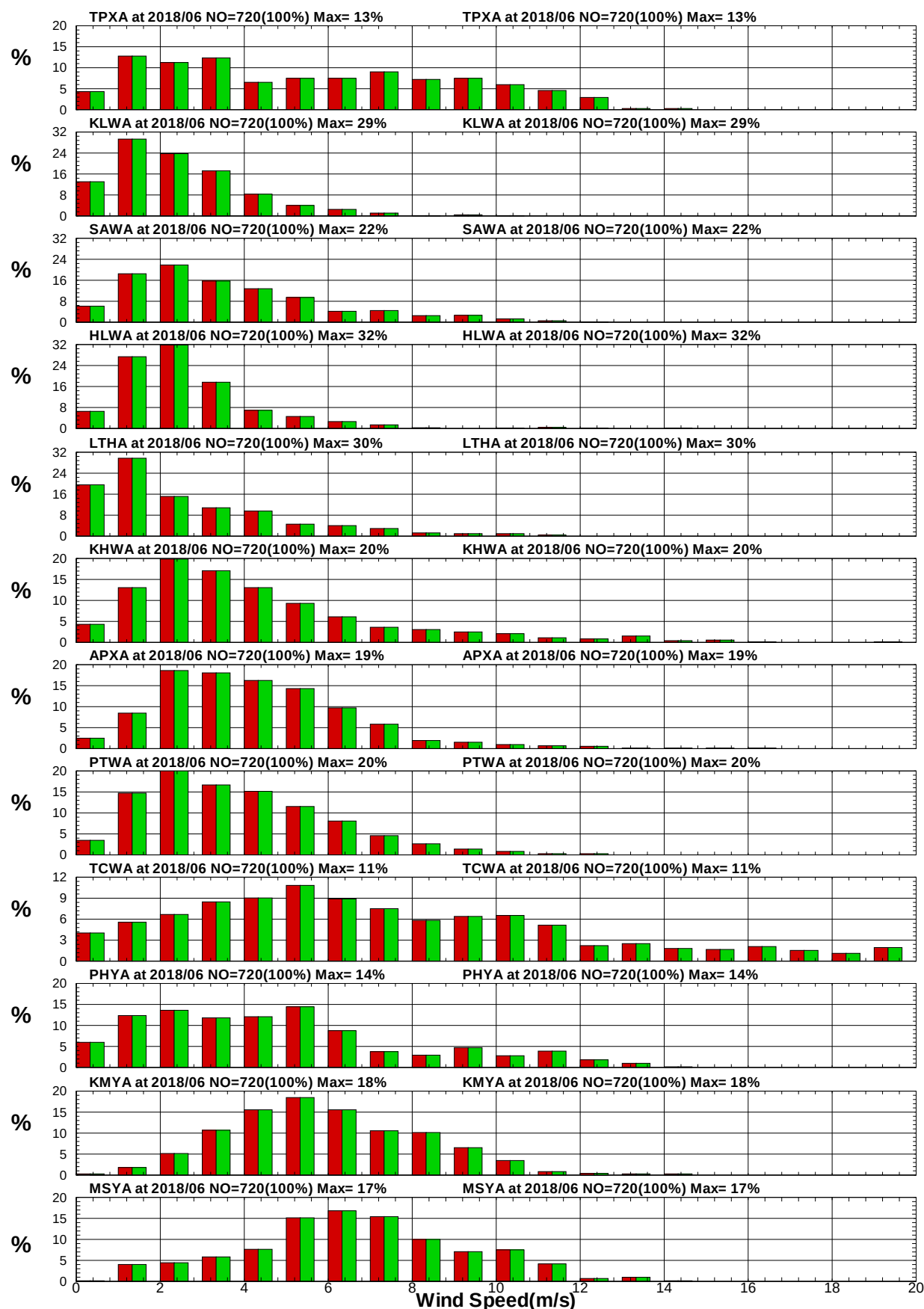
圖9.13 12港域2018年 6月 12月風速統計方塊圖
