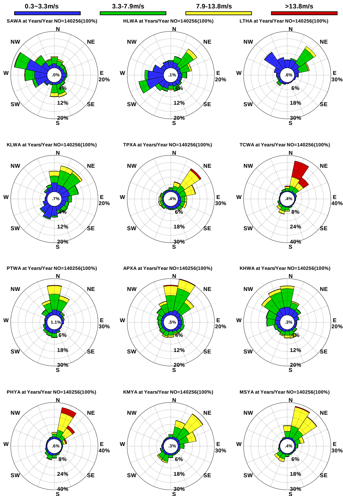
圖10.34 12港域歷年整年觀測風玫瑰比較圖
