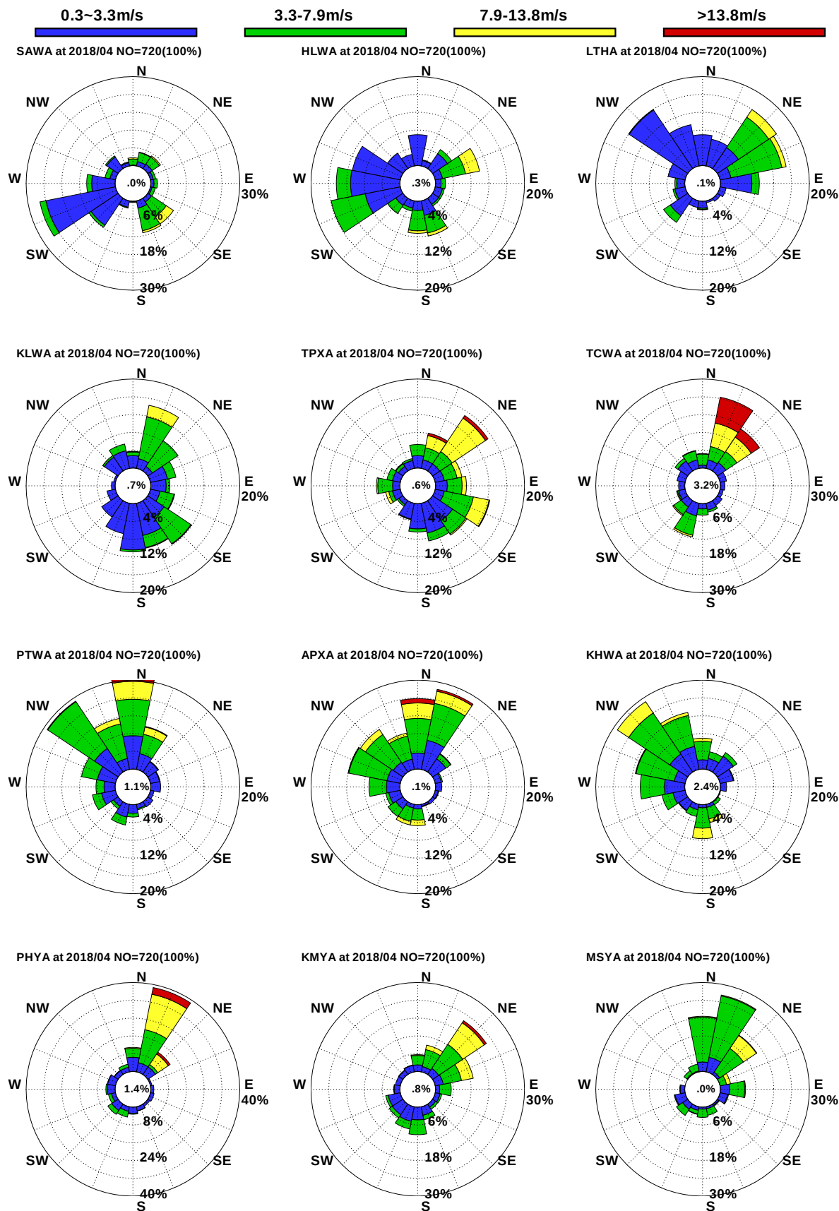
圖10.9 12港域2018年4月觀測風玫瑰比較圖
