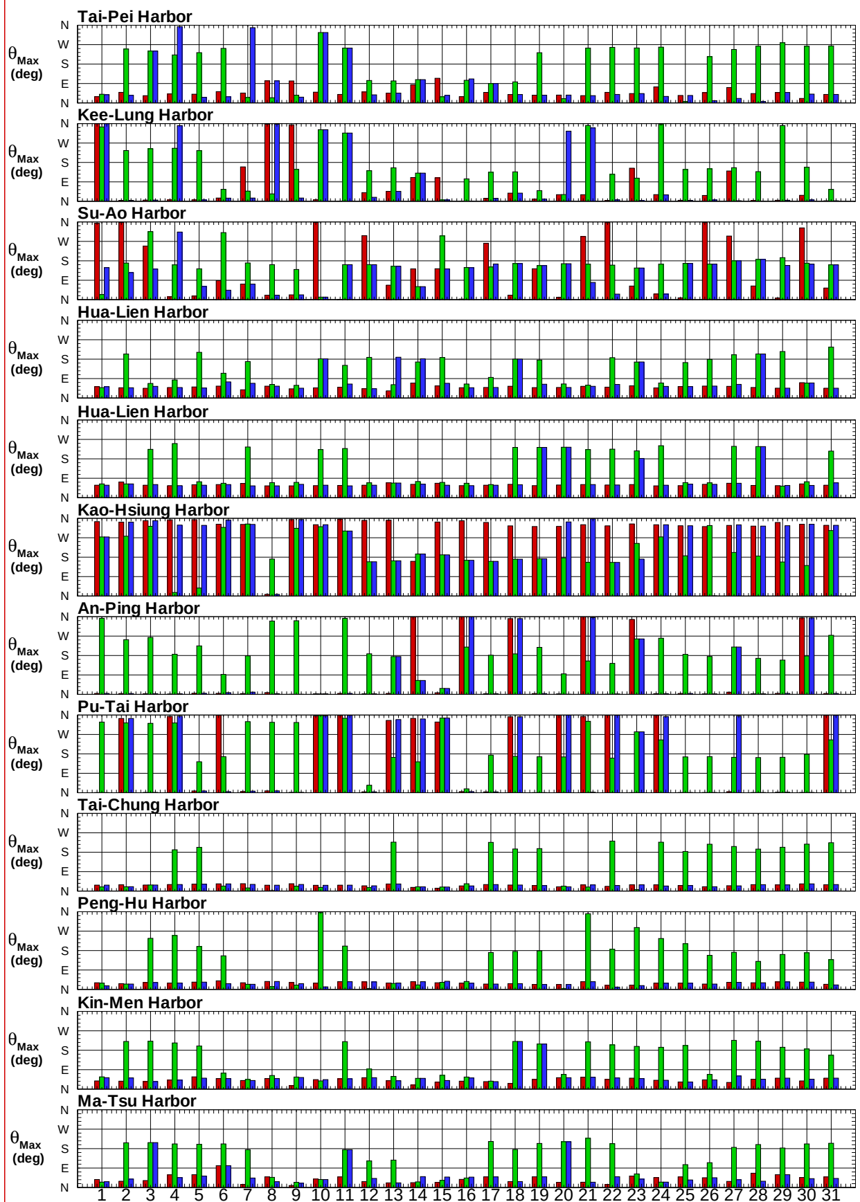
圖8.6d 2018年12港域冬, 夏及整年主要測站每日最大風速之風向圖
