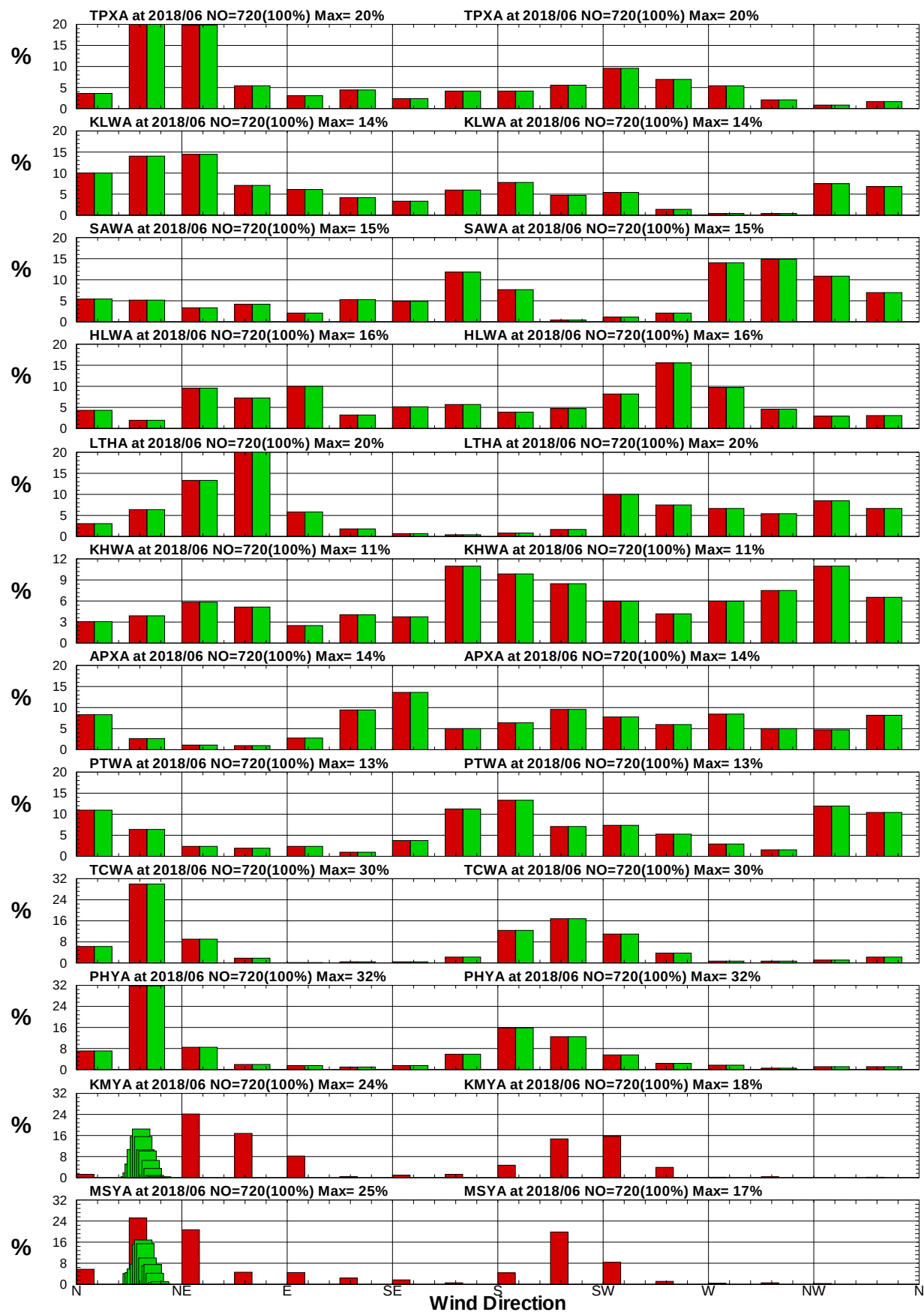
圖9.14 12港域2018年 6月年12月風向統計方塊圖
