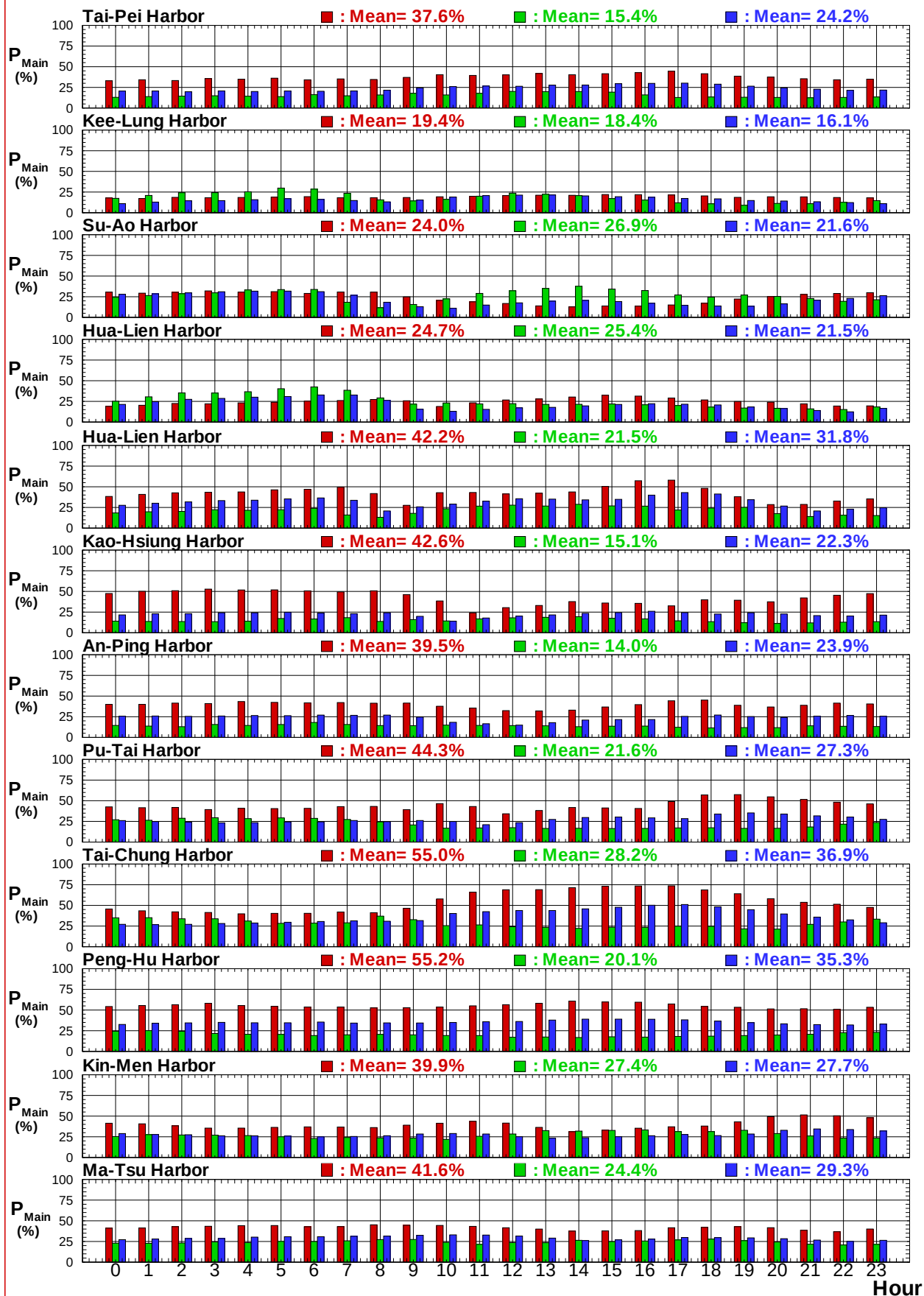
圖8.5f 歷年12港域冬, 夏及整年主要測站逐時主要風向百分比圖
