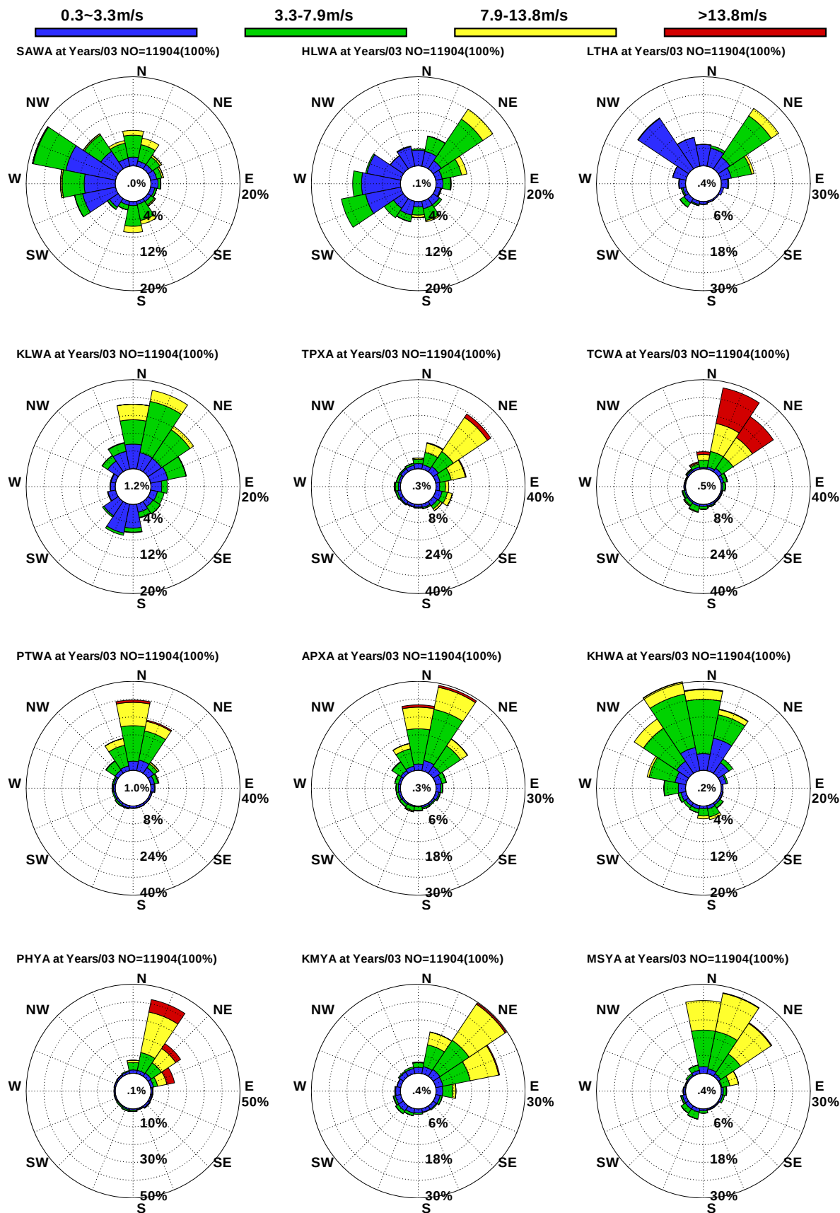
圖10.8 12港域歷年 3 月觀測風玫瑰比較圖
