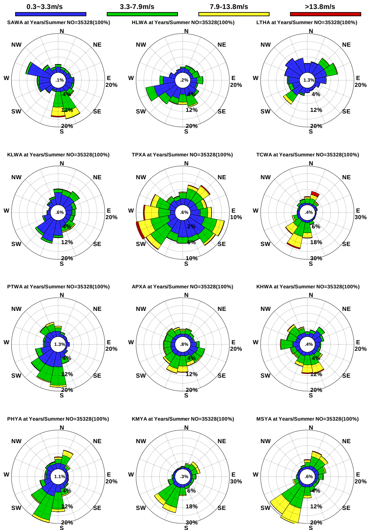
圖10.30 12港域歷年夏季觀測風玫瑰比較圖
