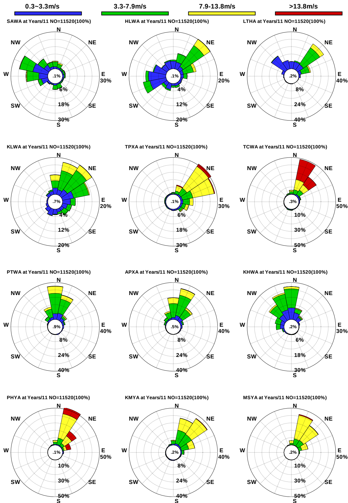
圖10.24 12港域歷年11月觀測風玫瑰比較圖
