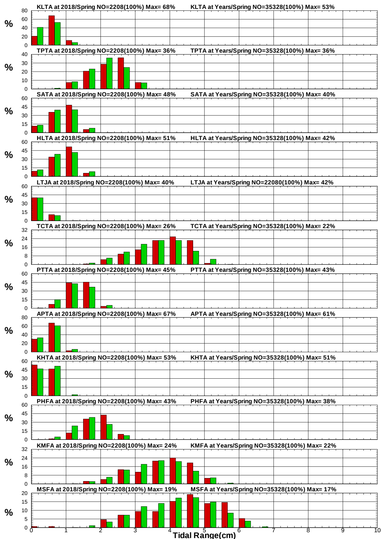
圖8.41 12港域2018年及歷年春季潮差統計方塊圖
