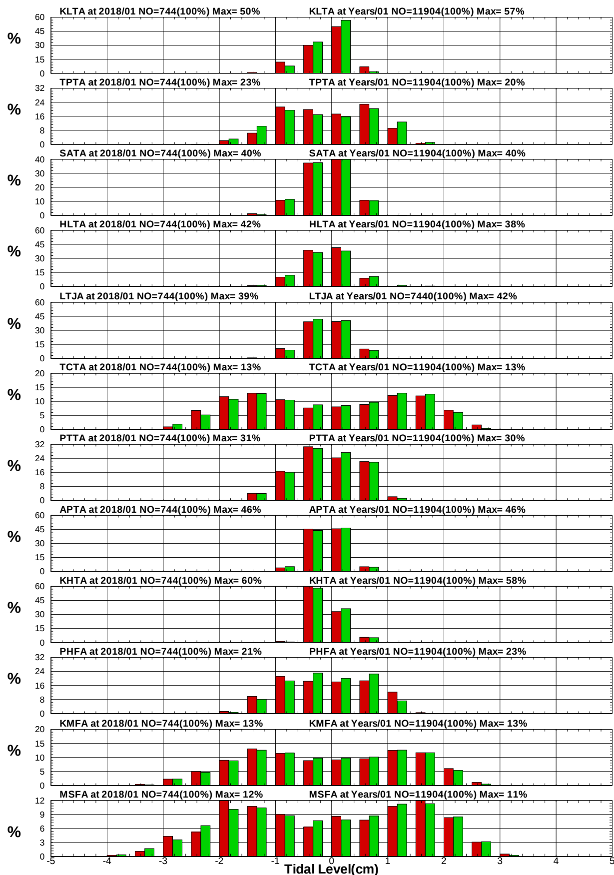
圖8.4 12港域2018年及歷年 1 月潮位統計方塊圖
