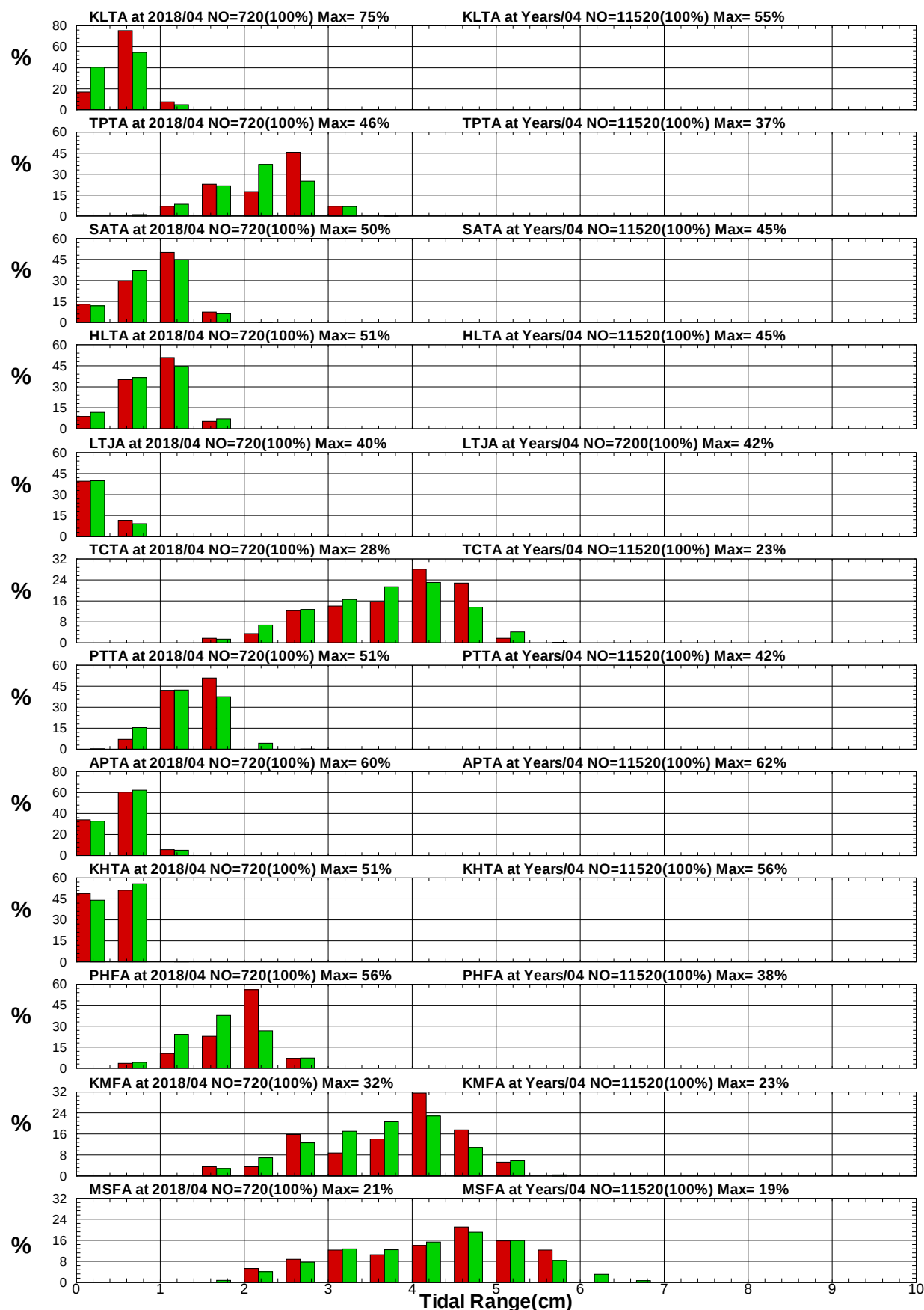
圖8.14 12港域2018年及歷年 4月潮差統計方塊圖
