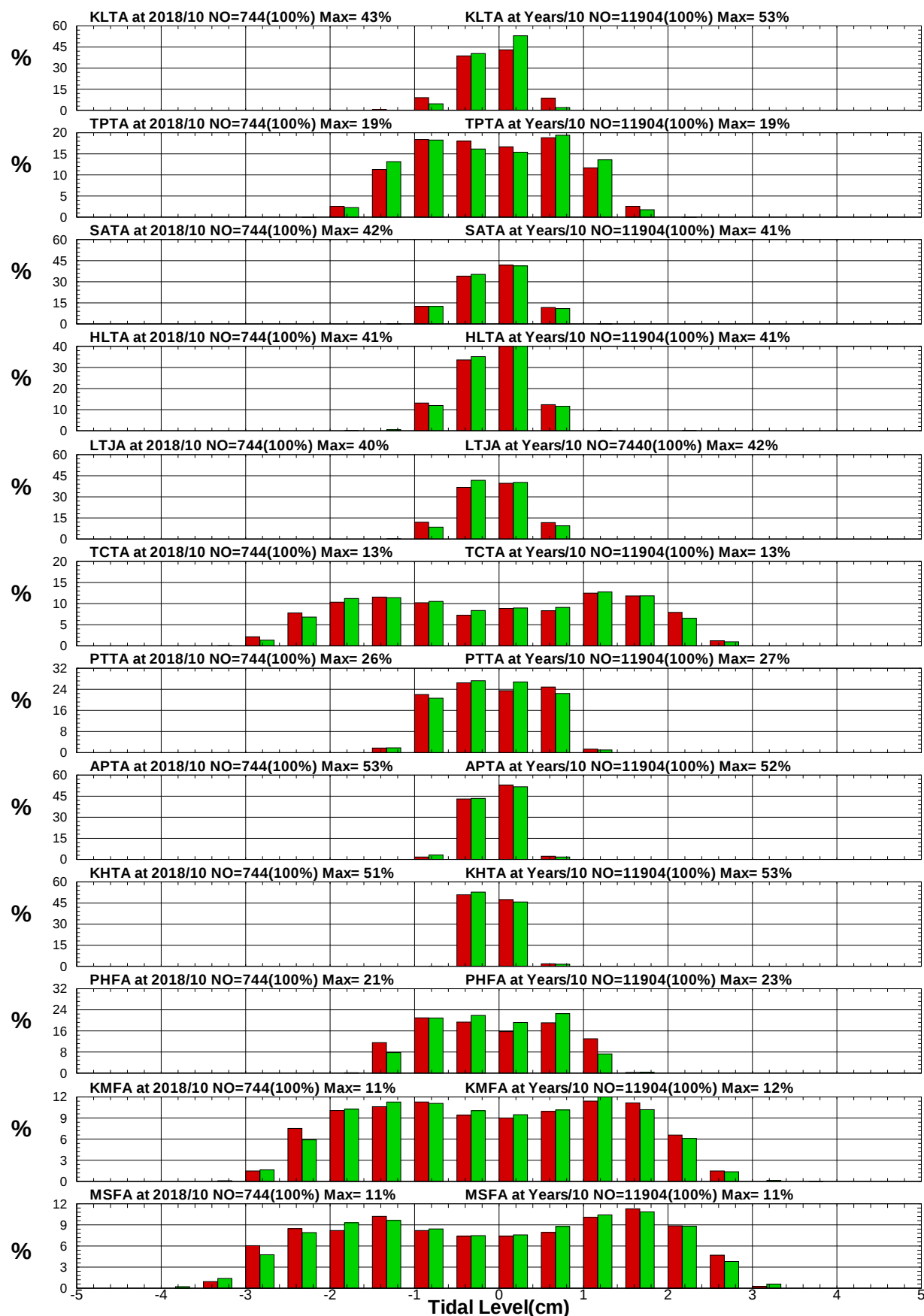
圖8.31 12港域2018年及歷年10月潮位統計方塊圖
