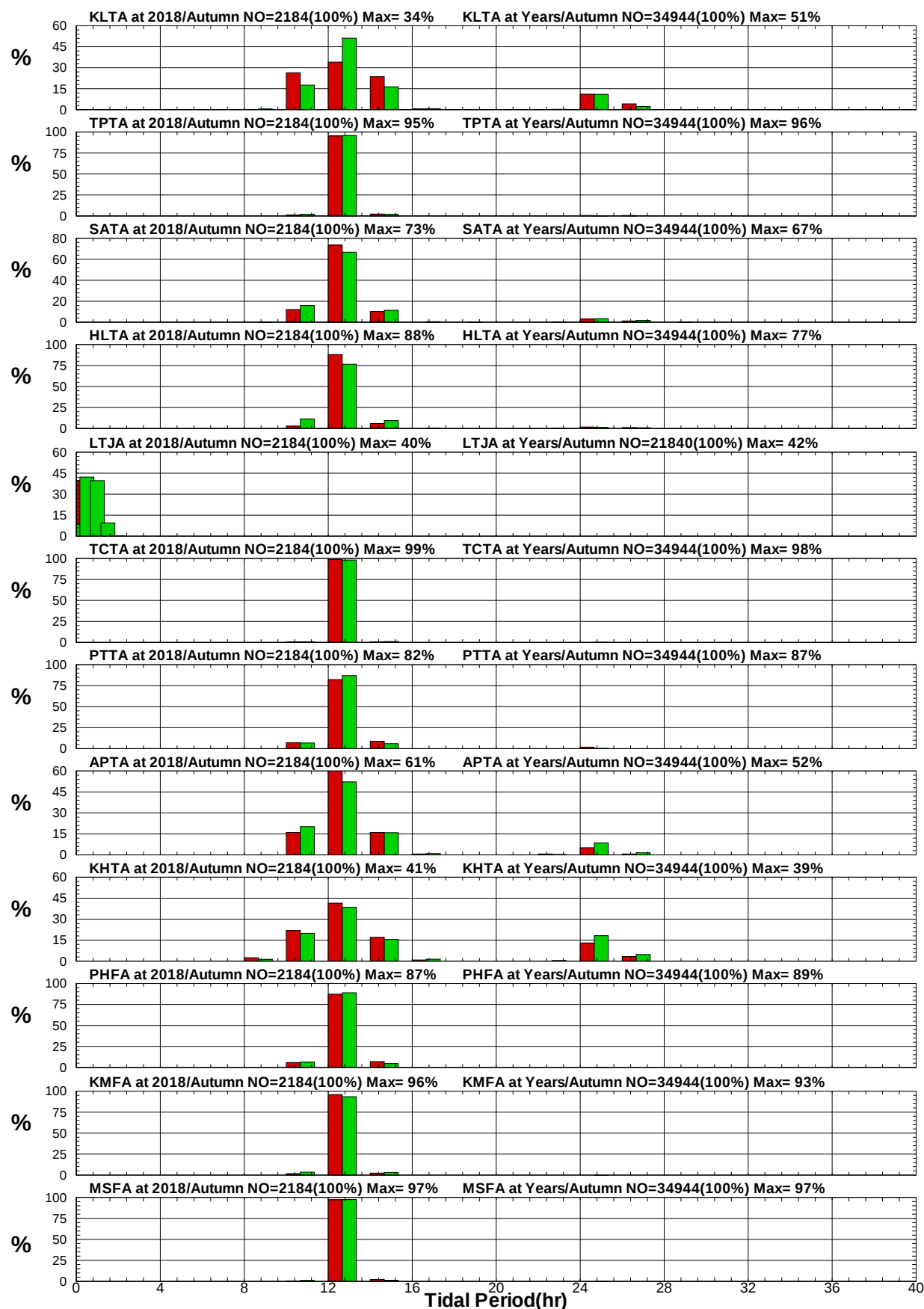
圖8.48 12港域2018年及歷年秋季週期統計方塊圖
