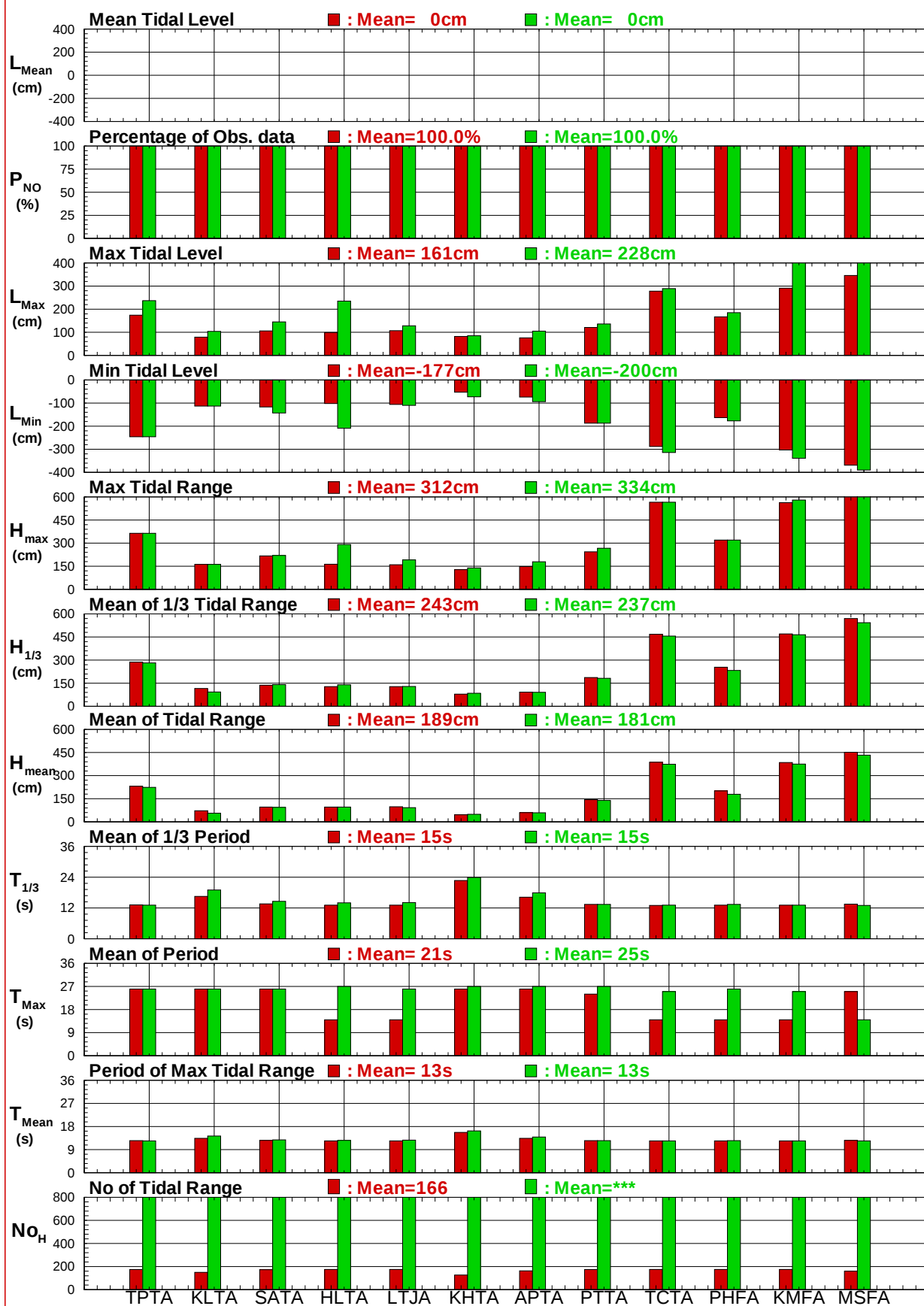
圖7.3 12個港域2018及歷年主要測站夏季潮位比較圖
