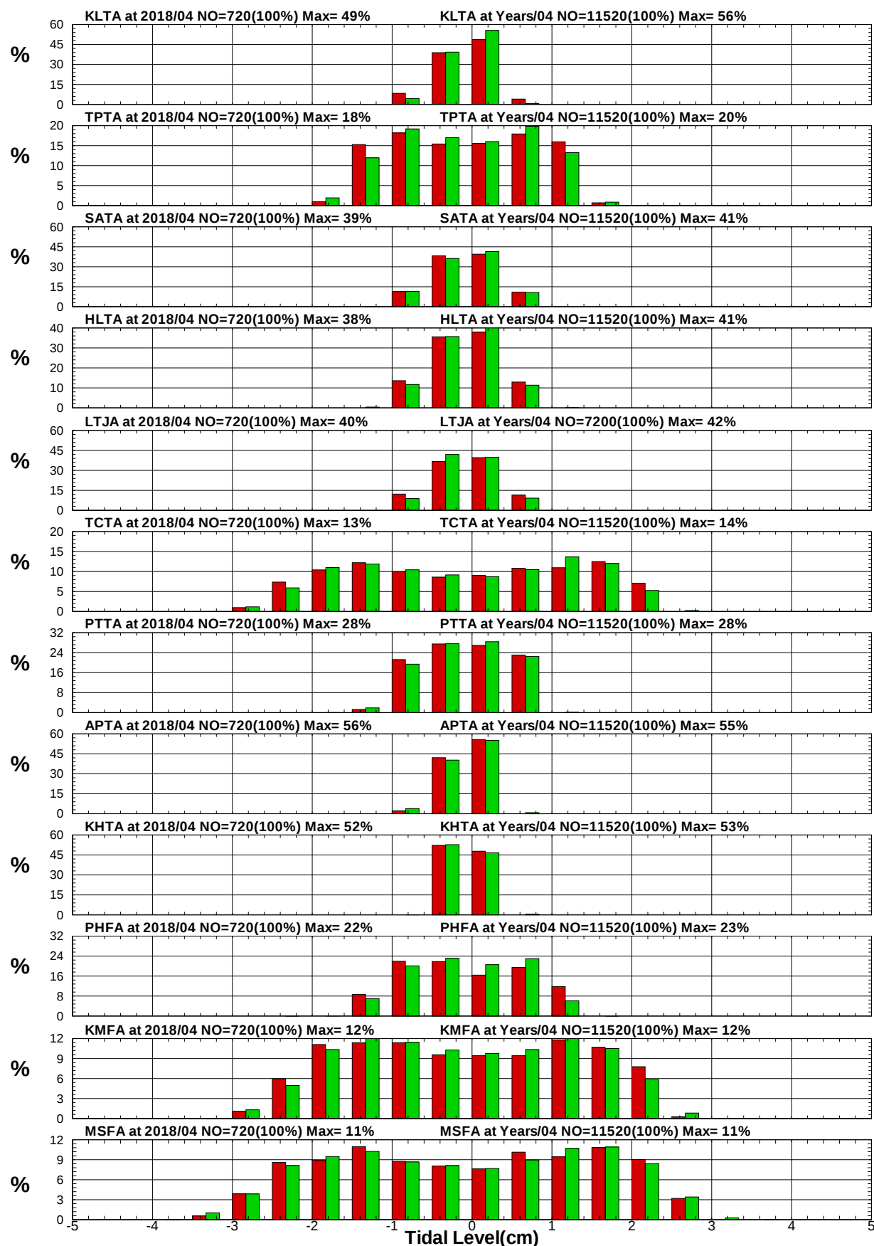
圖8.13 12港域2018年及歷年 4月潮位統計方塊圖
