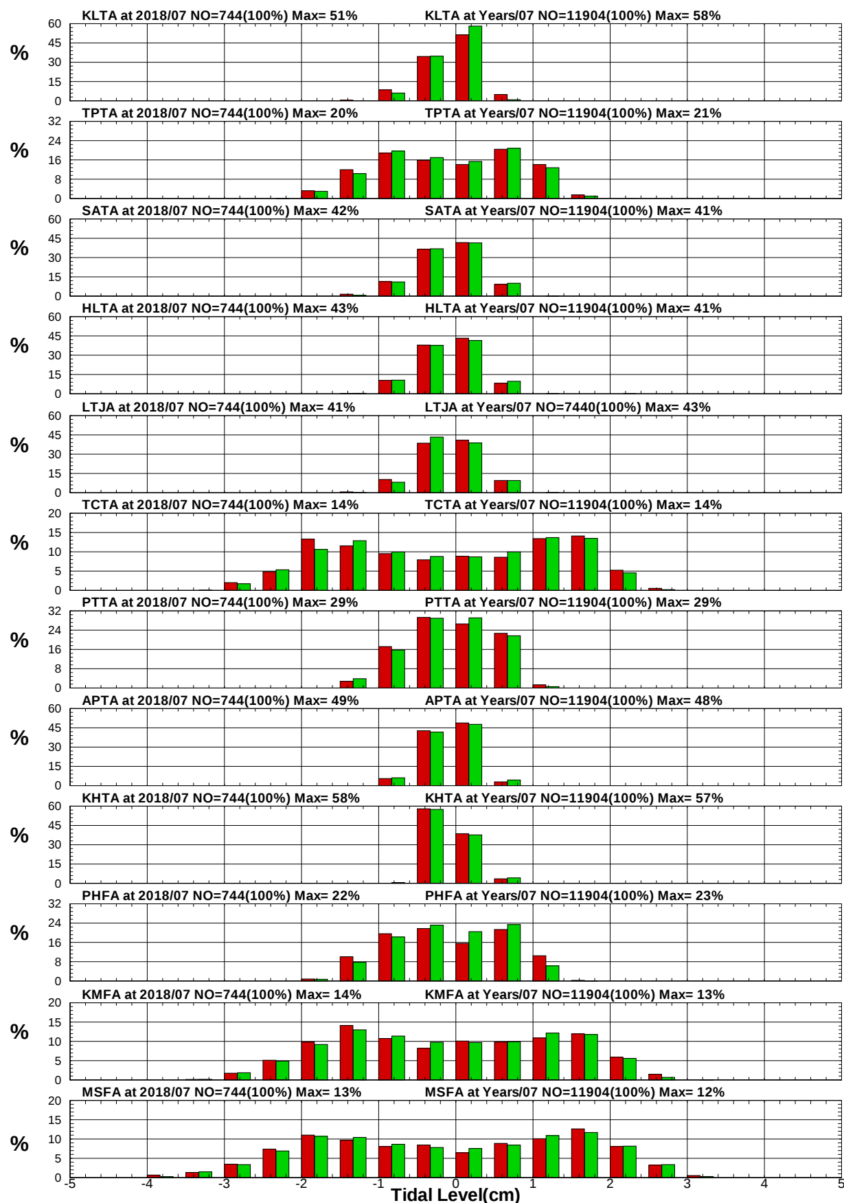
圖8.22 12港域2018年及歷年 7月潮位統計方塊圖
