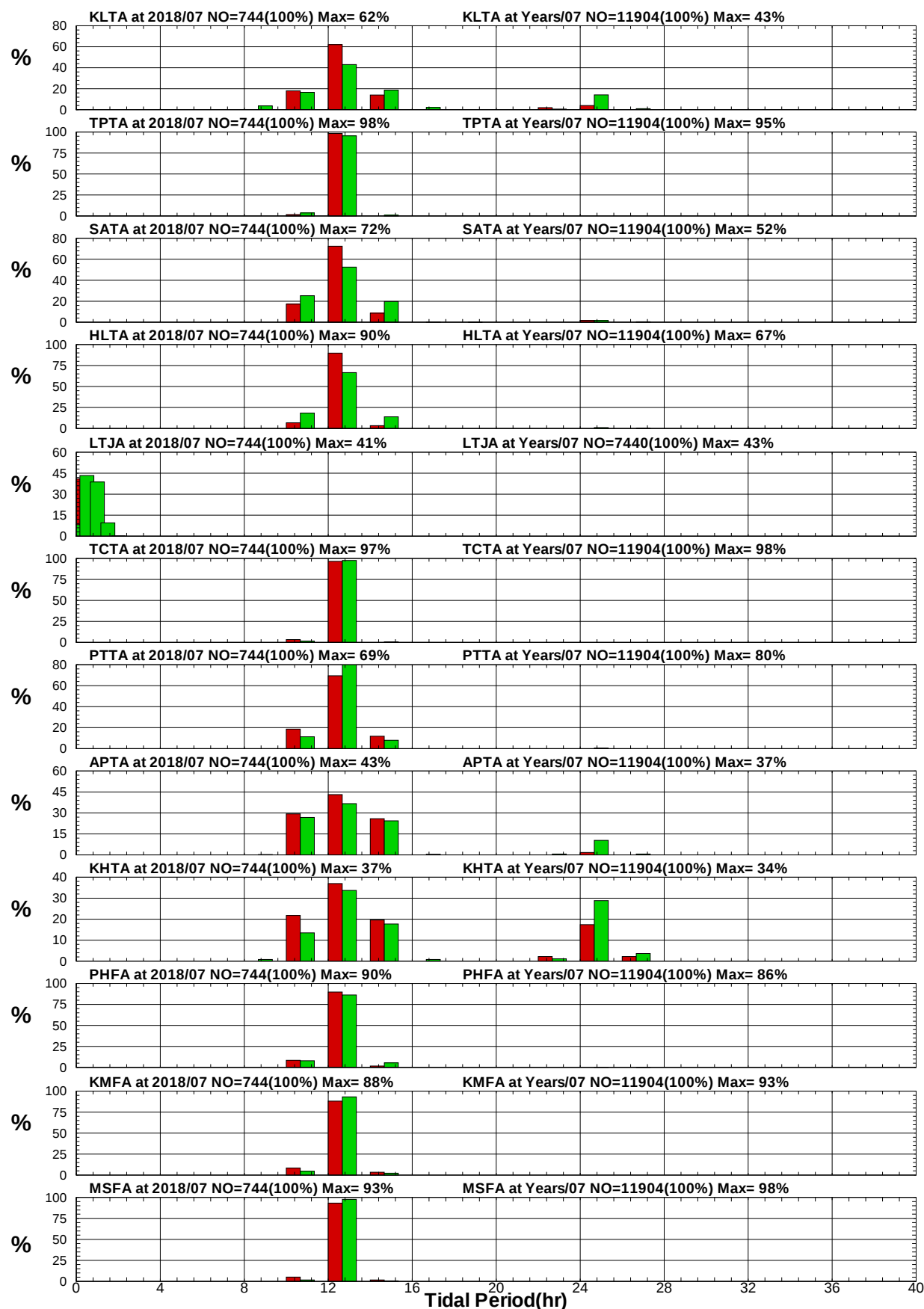
圖8.24 12港域2018年及歷年 7月週期統計方塊圖
