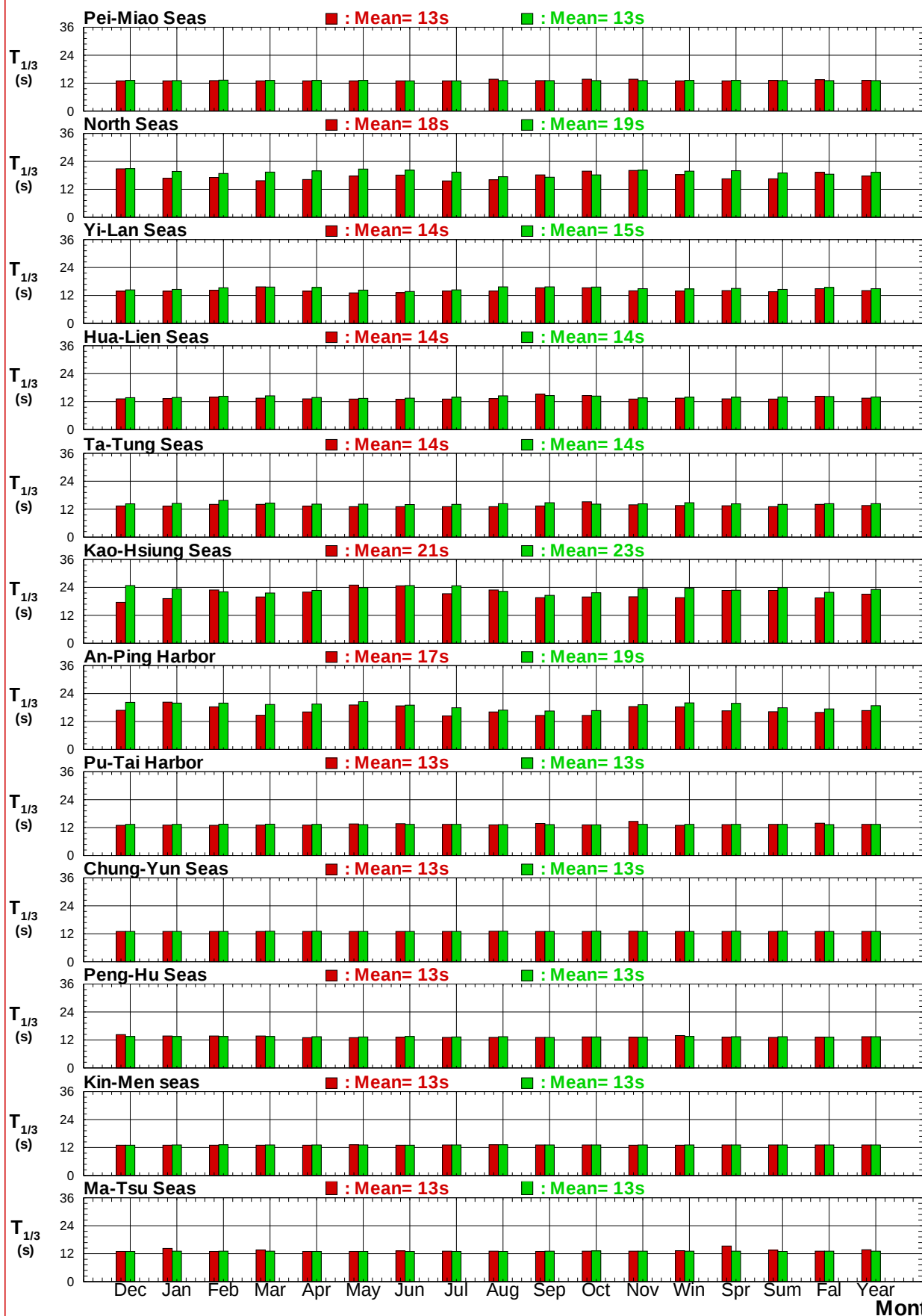
圖7.17 12個港域2018及歷年主要測站每月(季) 1/3週期比較圖
