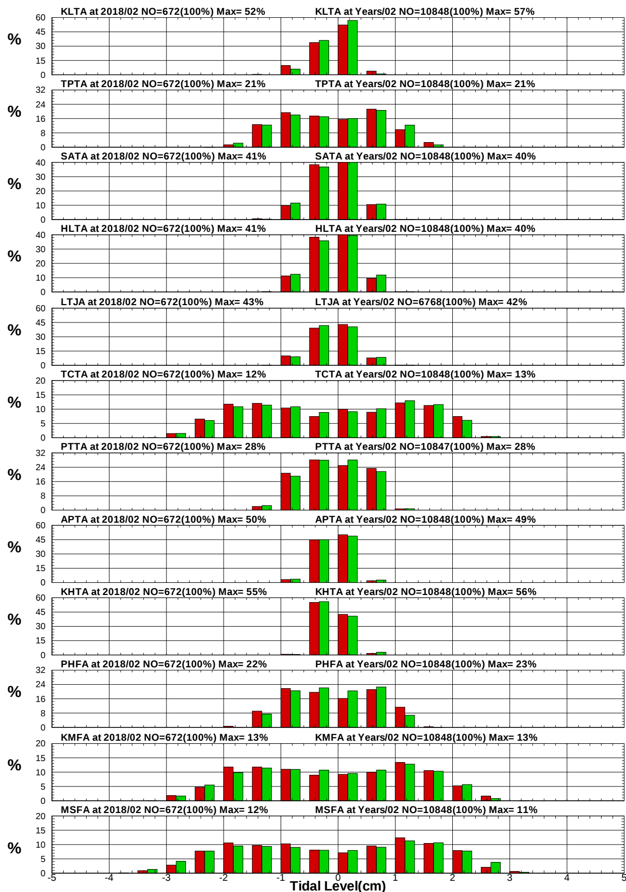
圖8.7 12港域2018年及歷年 2月潮位統計方塊圖
