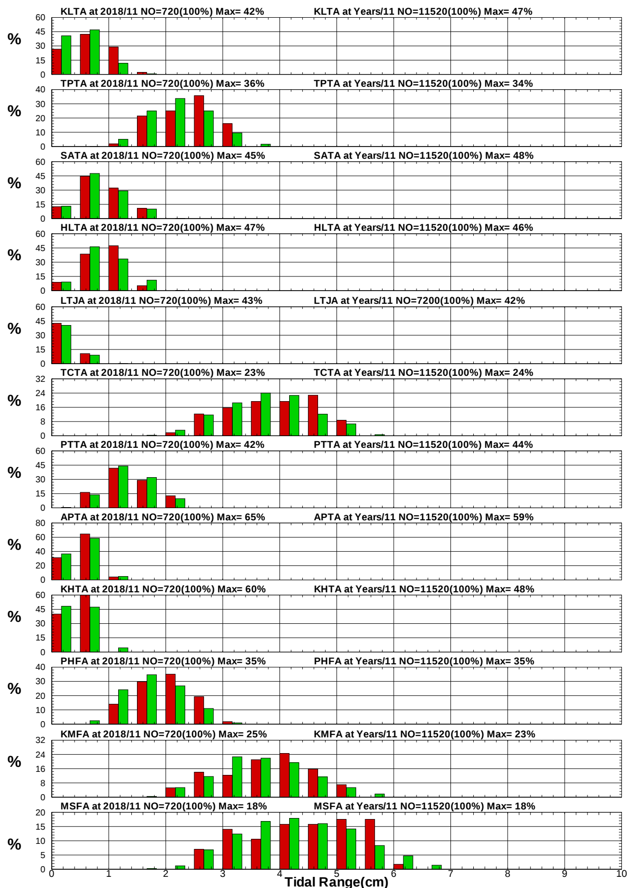
圖8.35 12港域2018年及歷年11月潮差統計方塊圖
