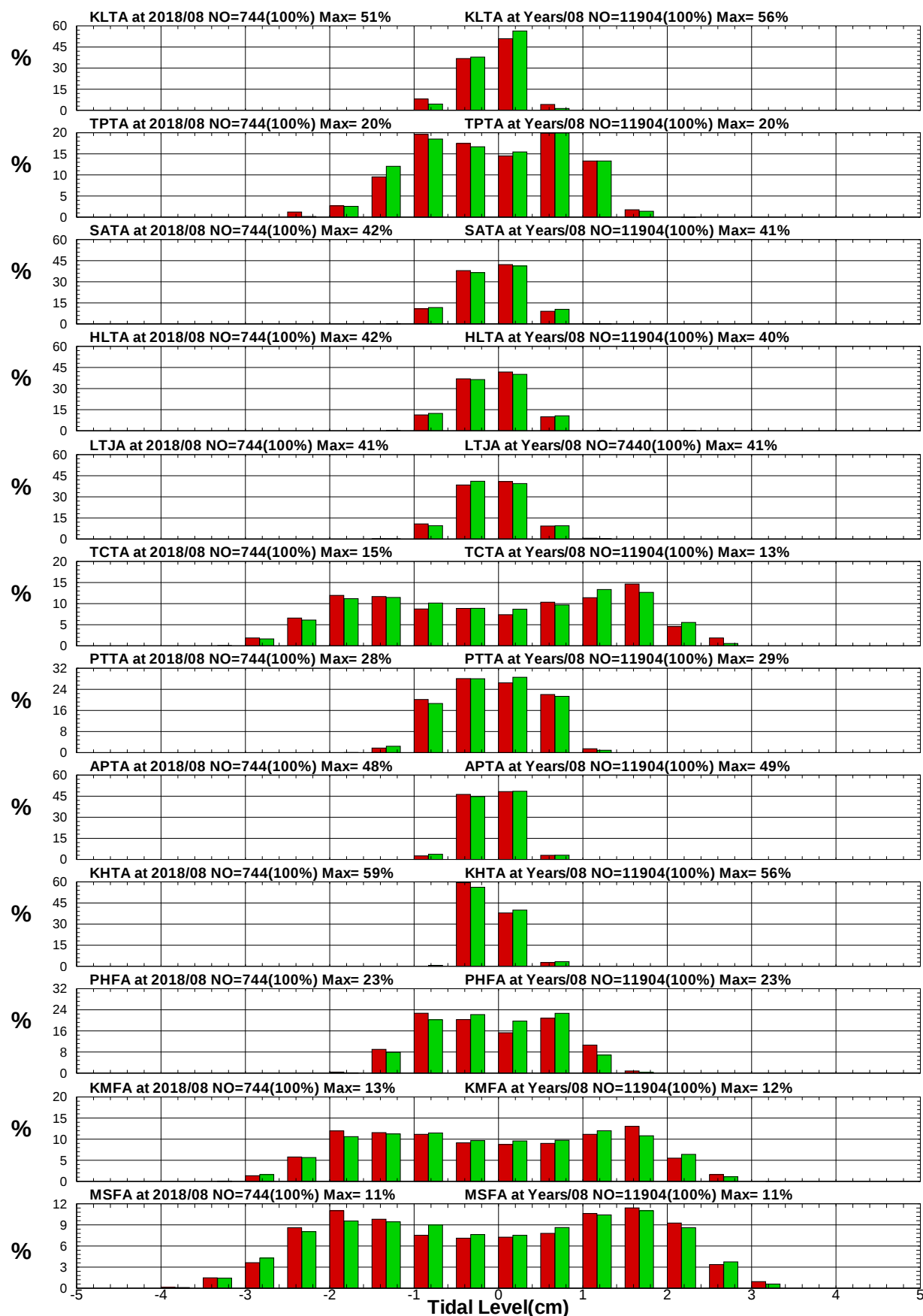
圖8.25 12港域2018年及歷年 8 月潮位統計方塊圖
