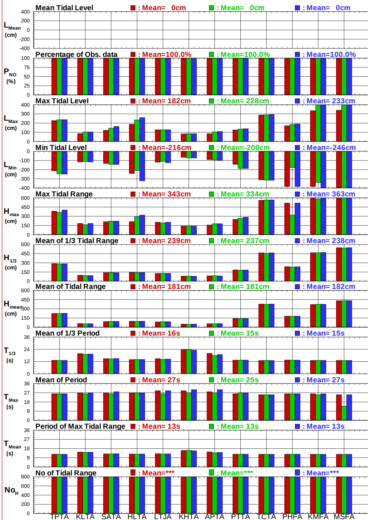
圖7.7 12個港域歷年主要測站冬, 夏及整年潮位比較圖
