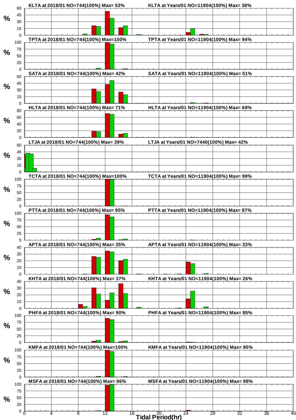
圖8.6 12港域2018年及歷年 1 月週期統計方塊圖
