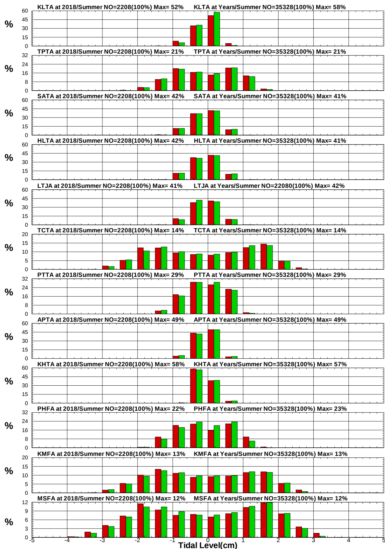
圖8.43 12港域2018年及歷年夏季潮位統計方塊圖
