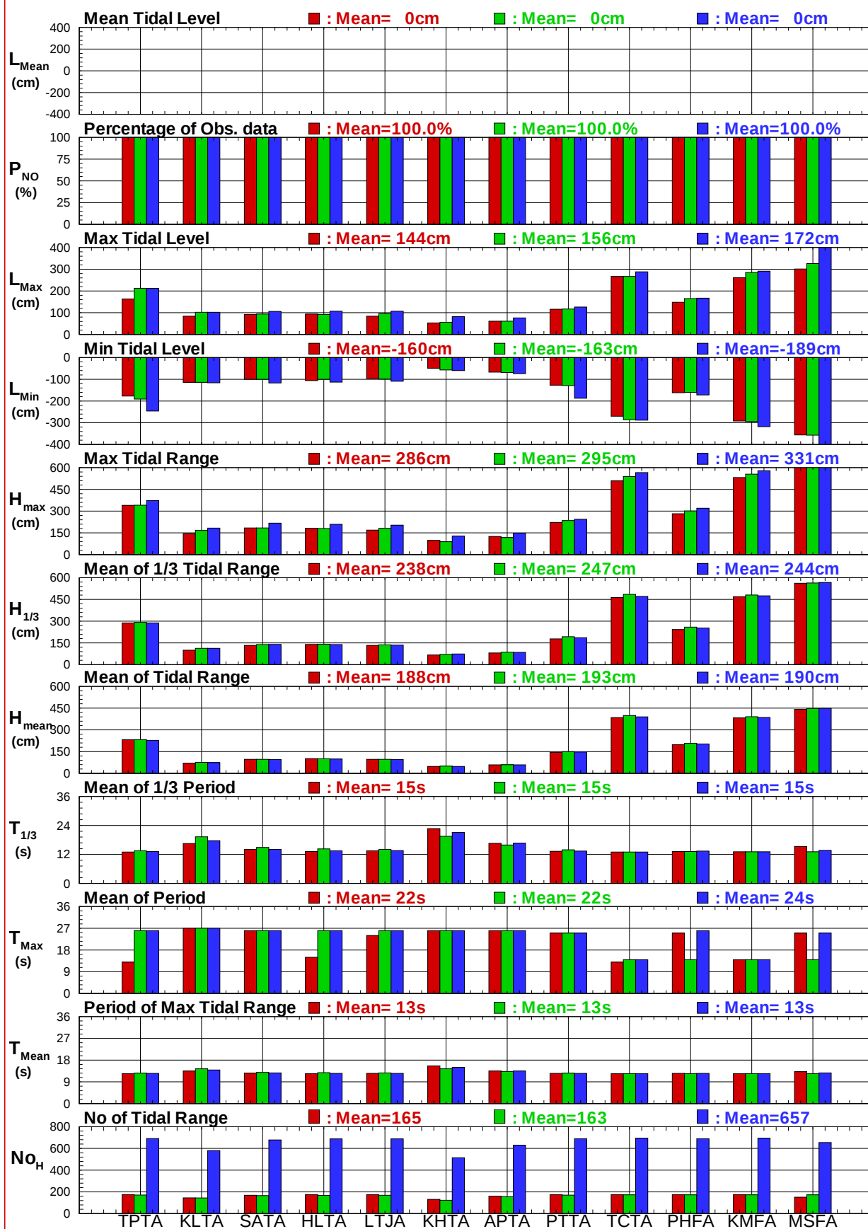
圖7.8 12個港域2018年主要測站春, 秋及整年潮位比較圖
