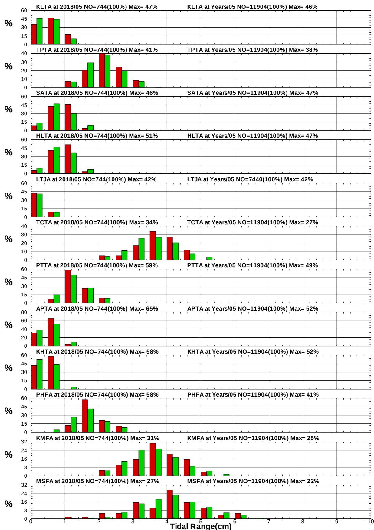
圖8.17 12港域2018年及歷年5月潮差統計方塊圖
