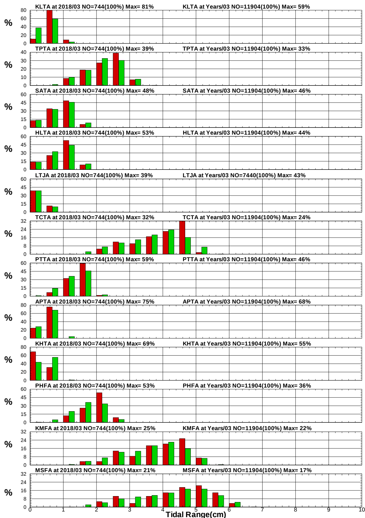
圖8.11 12港域2018年及歷年 3月潮差統計方塊圖
