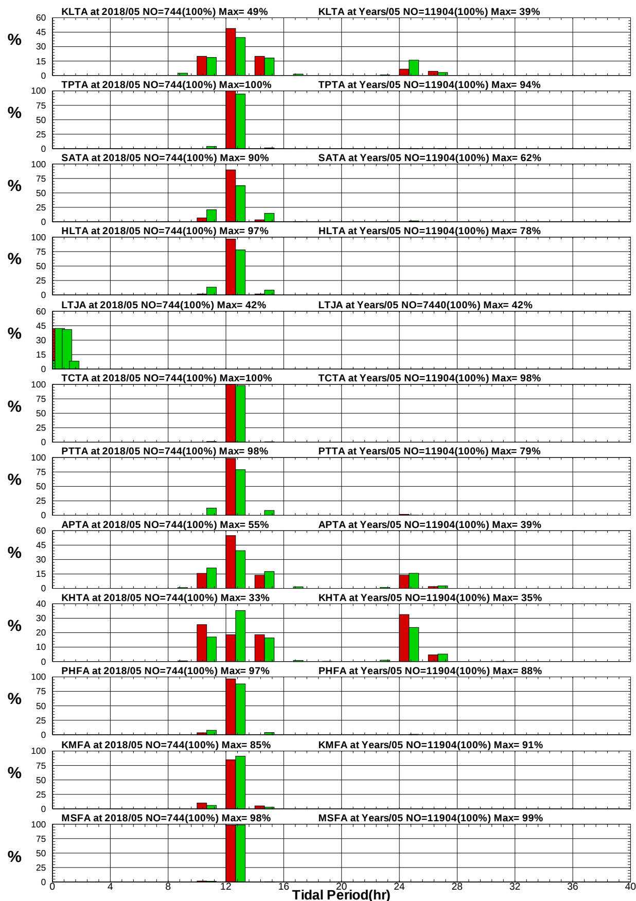
圖8.18 12港域2018年及歷年 5月週期統計方塊圖
