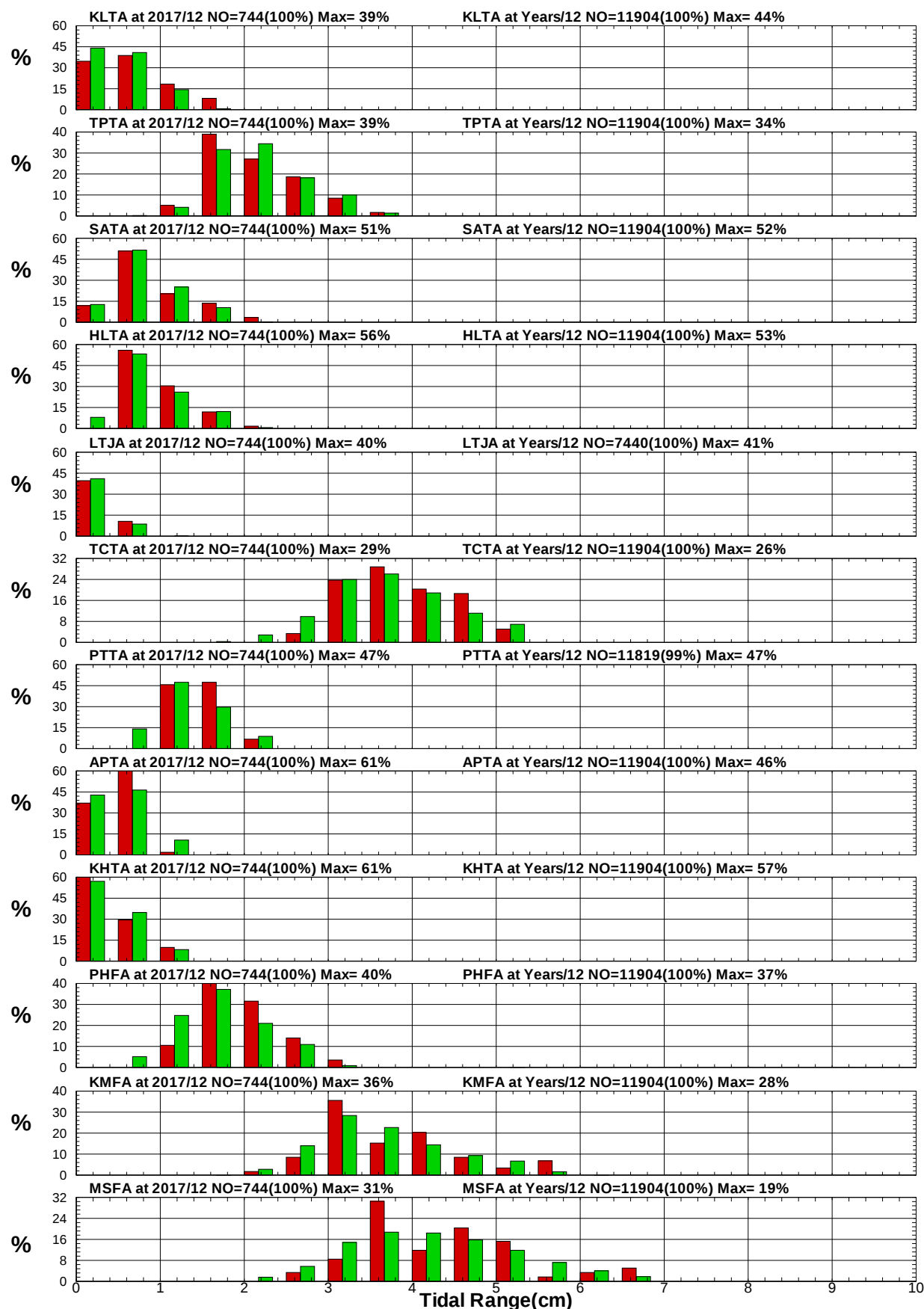
圖8.2 12港域2017年及歷年12月潮差統計方塊圖
