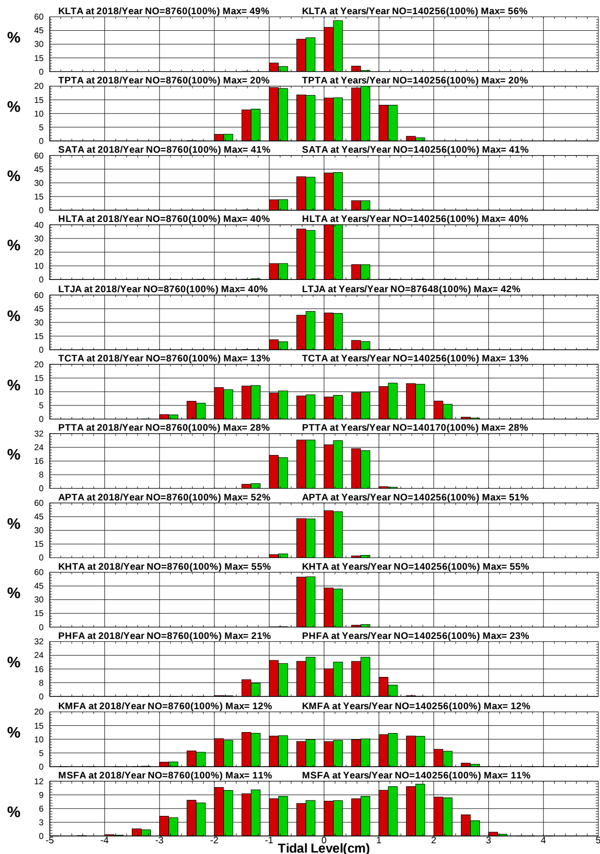
圖8.49 12港域2018年及歷年整年潮位統計方塊圖
