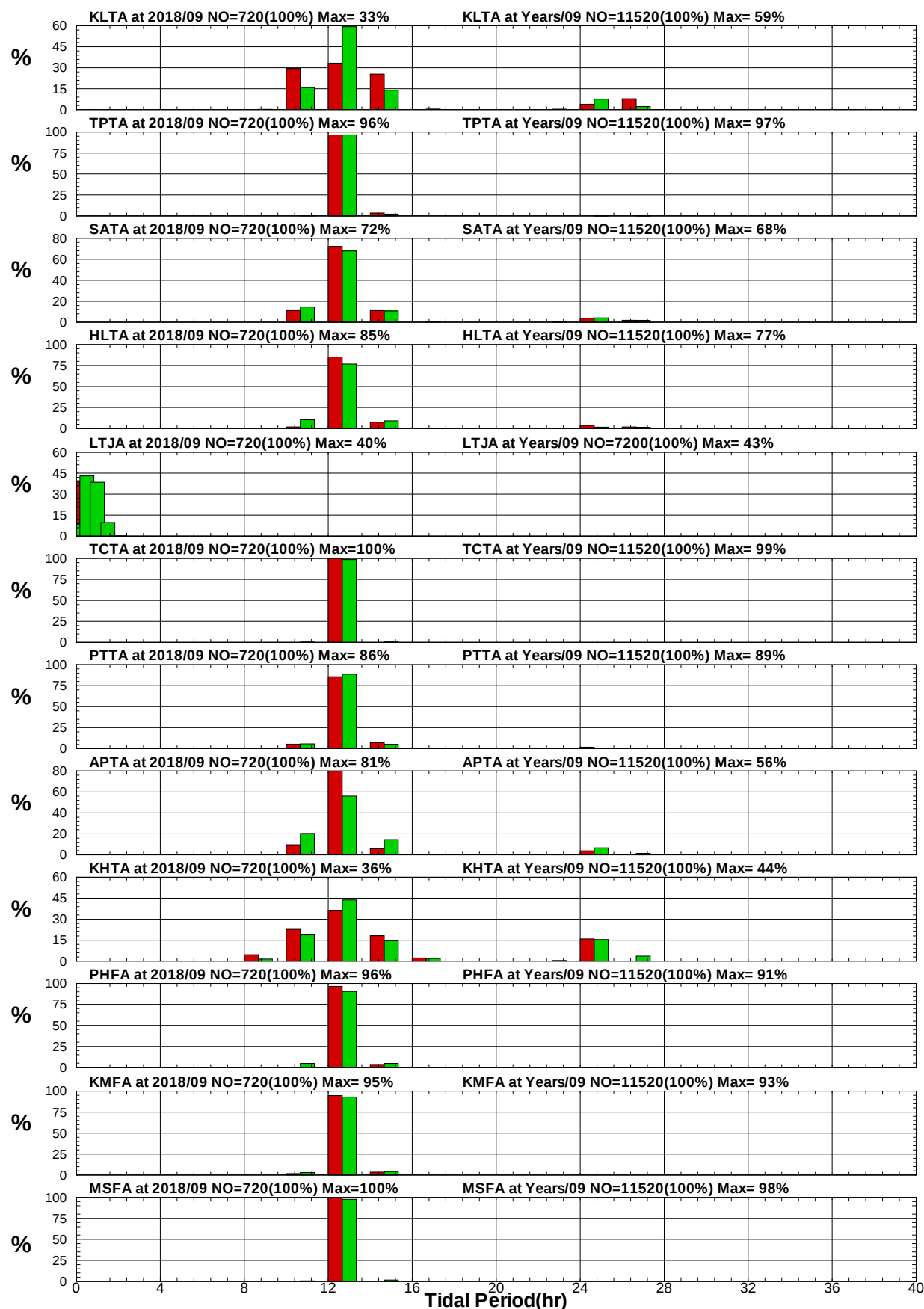
圖8.30 12港域2018年及歷年 9 月週期統計方塊圖
