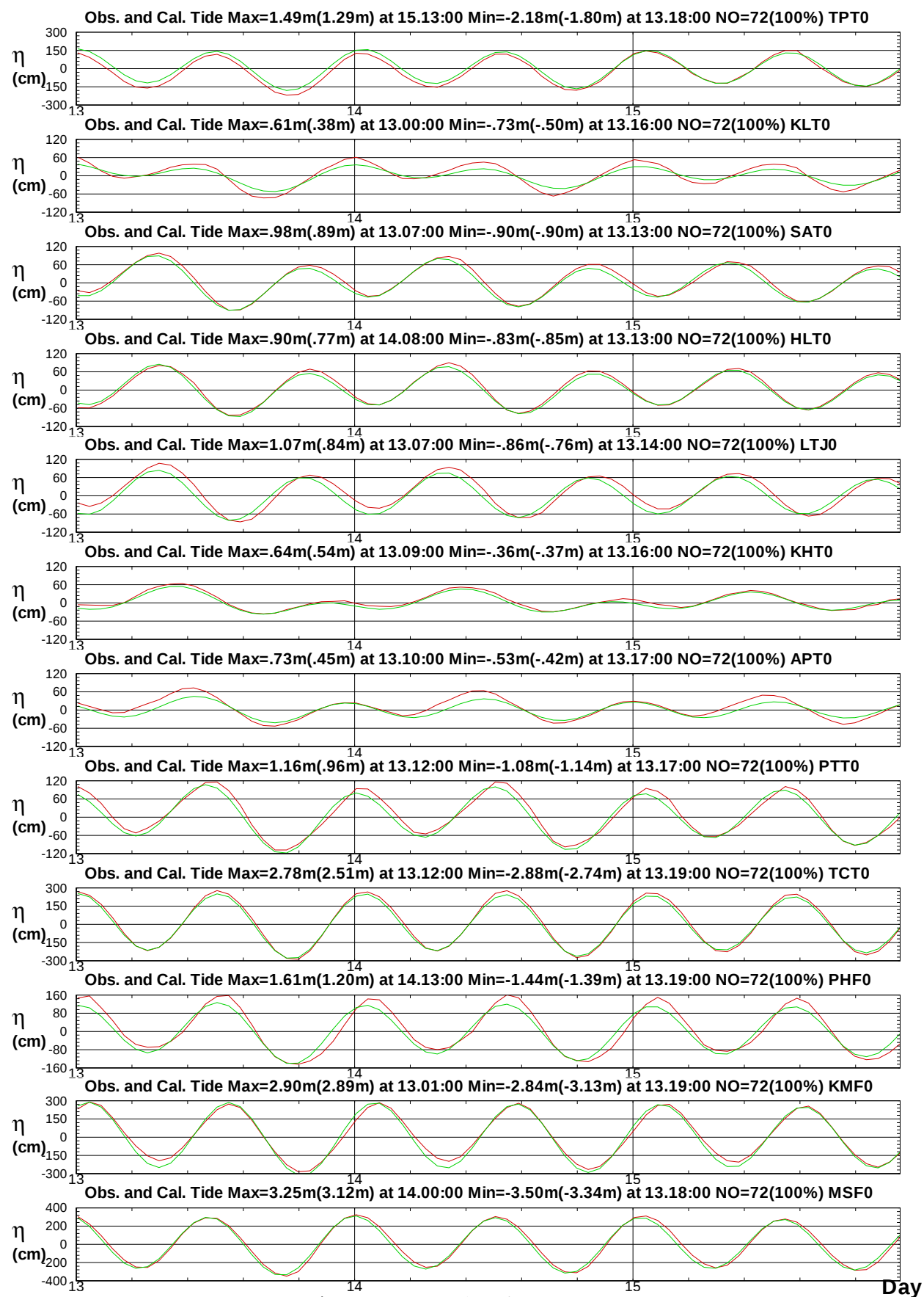
圖9.2 2018年山竹 颱風12海域觀測潮位歷線圖 (細: 天文潮)
