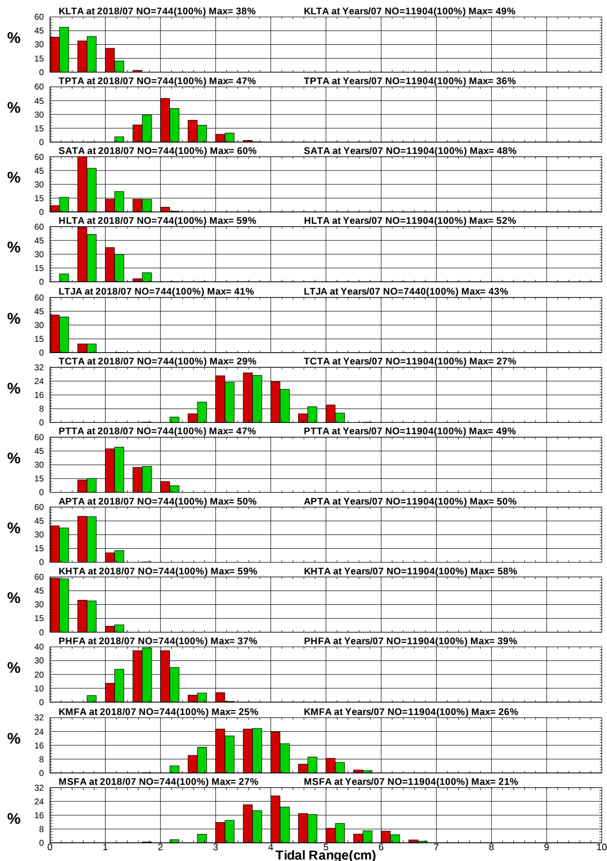
圖8.23 12港域2018年及歷年 7月潮差統計方塊圖
