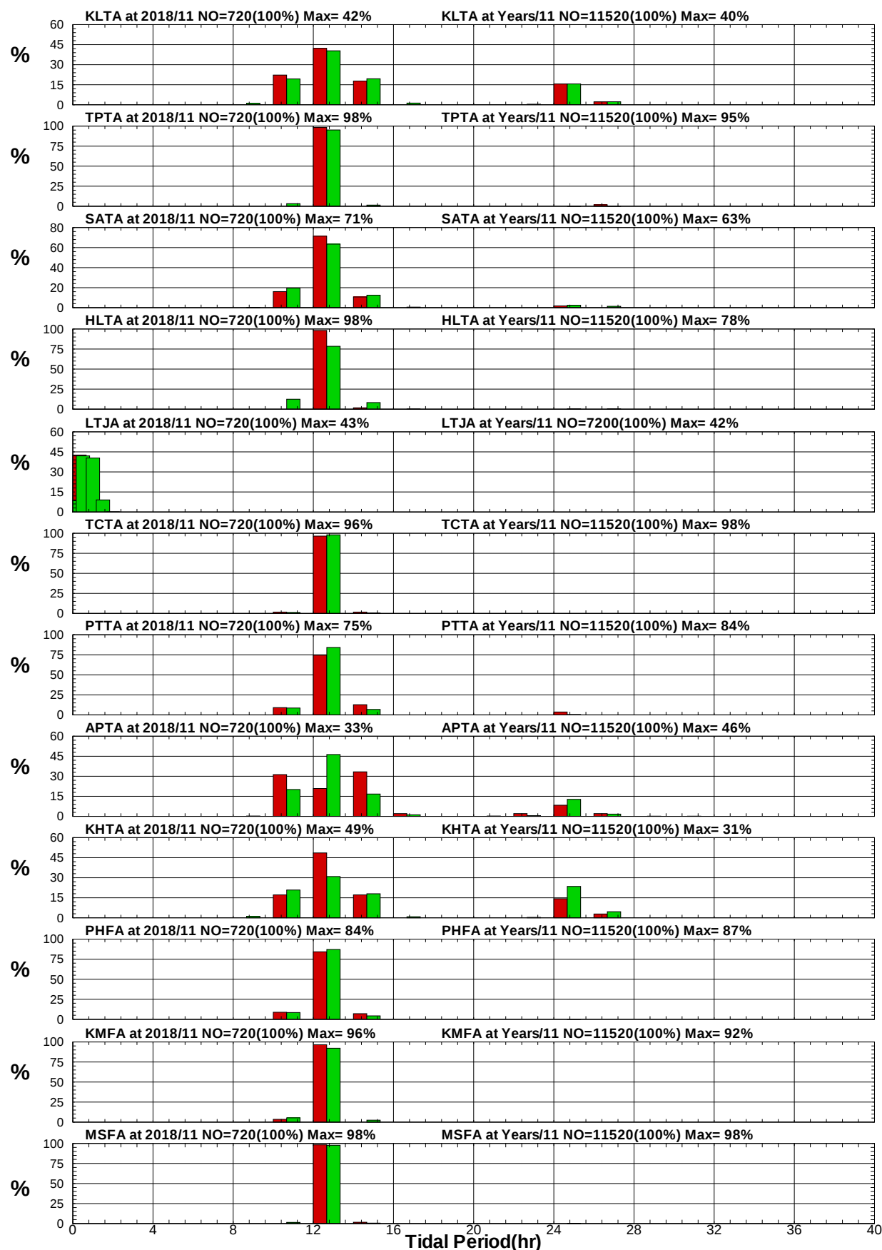
圖8.36 12港域2018年及歷年11月週期統計方塊圖
