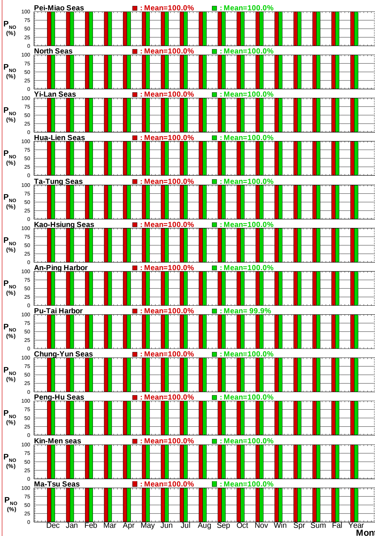
圖7.11 12個港域2018及歷年主要測站每月(季)潮位資料蒐集率比較圖
