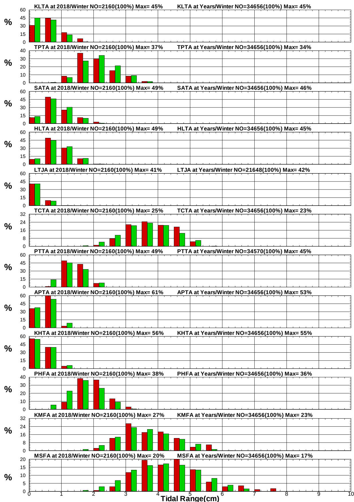
圖8.38 12港域2018年及歷年冬季潮差統計方塊圖
