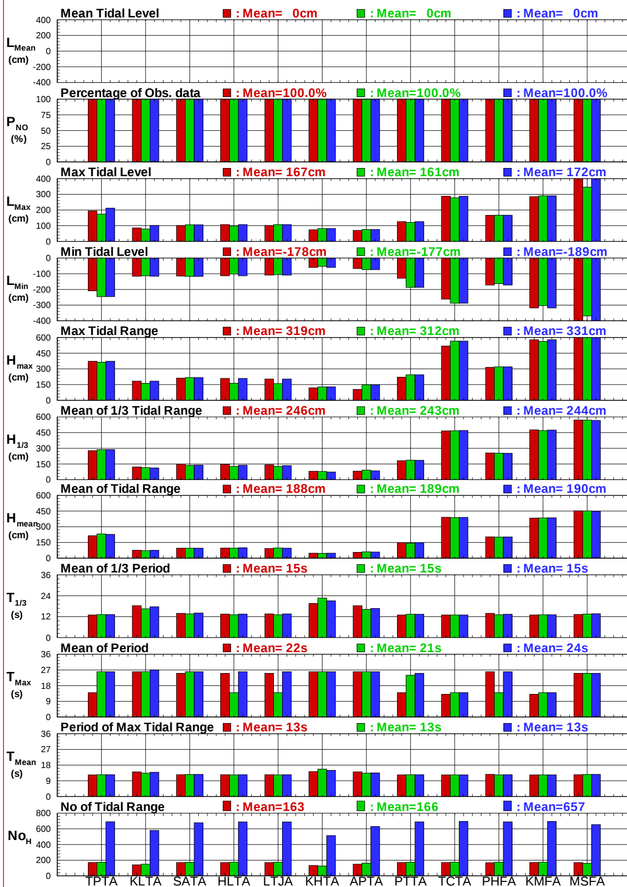
圖7.6 12個港域2018年主要測站冬、夏及整年潮位比較圖
