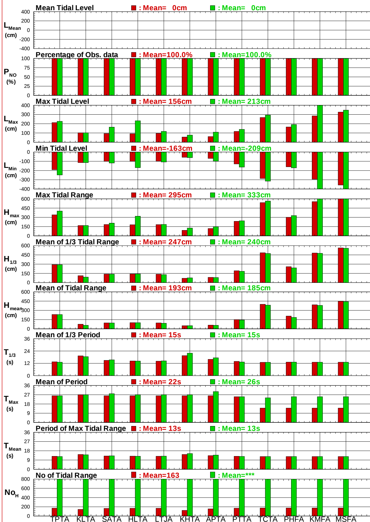
圖7.4 12個港域2018及歷年主要測站秋季潮位比較圖
