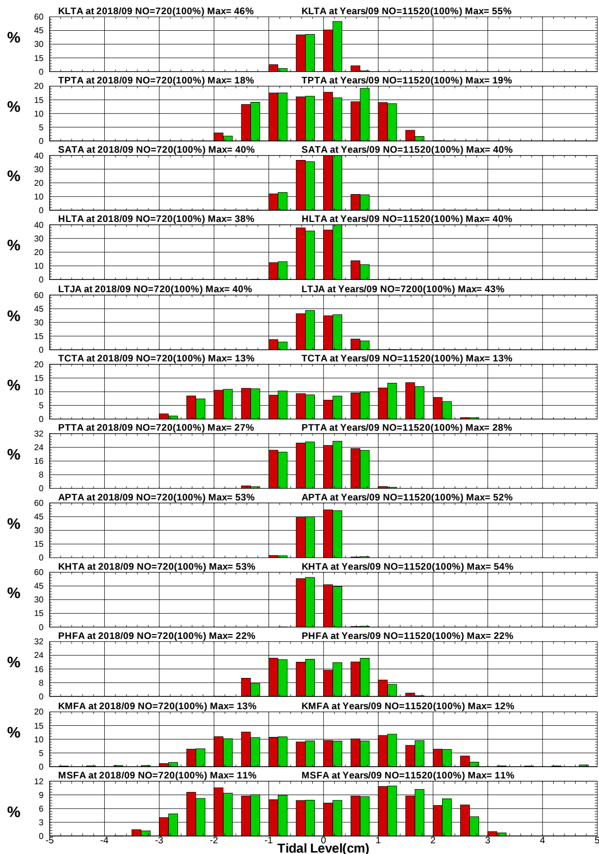
圖8.28 12港域2018年及歷年 9 月潮位統計方塊圖
