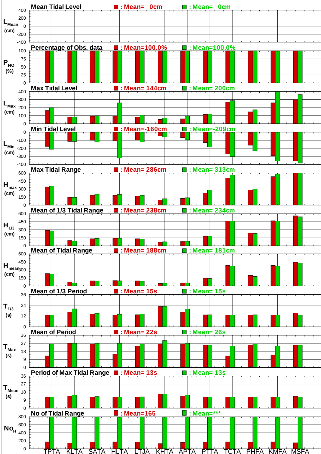
圖7.2 12個港域2018及歷年主要測站春季潮位比較圖
