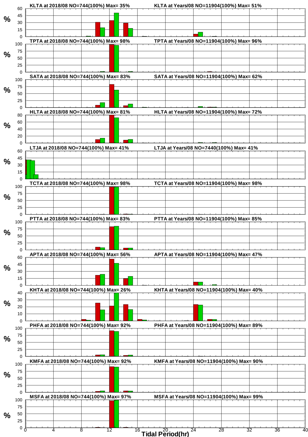
圖8.27 12港域2018年及歷年 8 月週期統計方塊圖
