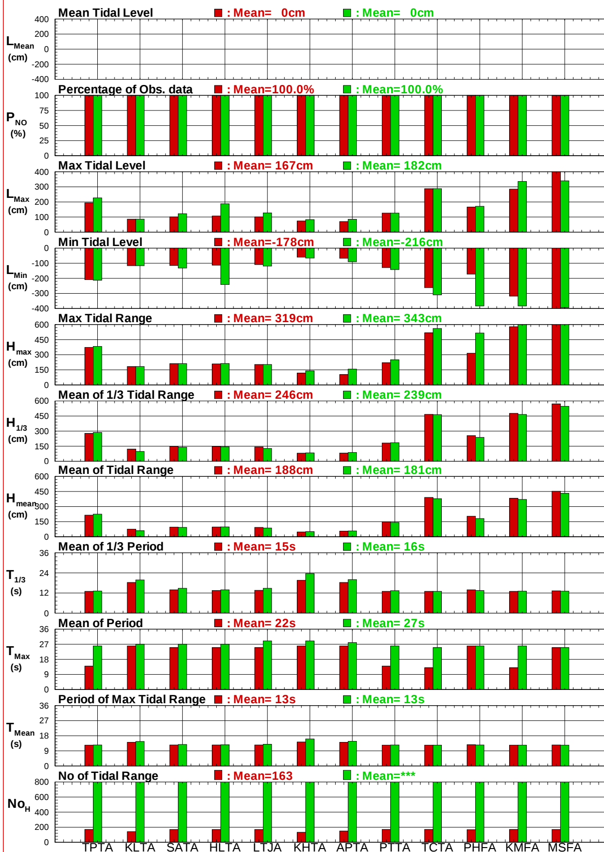
圖7.1 12個港域2018及歷年主要測站冬季潮位比較圖
