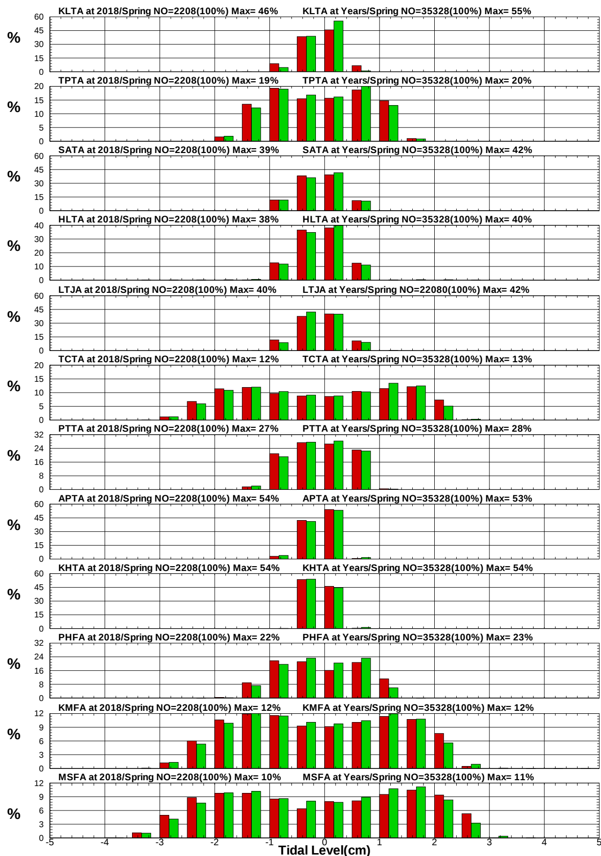
圖8.40 12港域2018年及歷年春季潮位統計方塊圖
