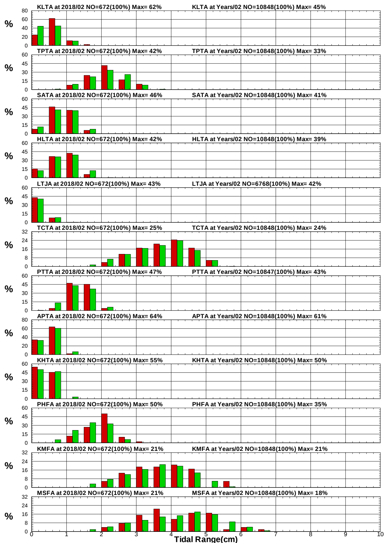
圖8.8 12港域2018年及歷年 2月潮差統計方塊圖
