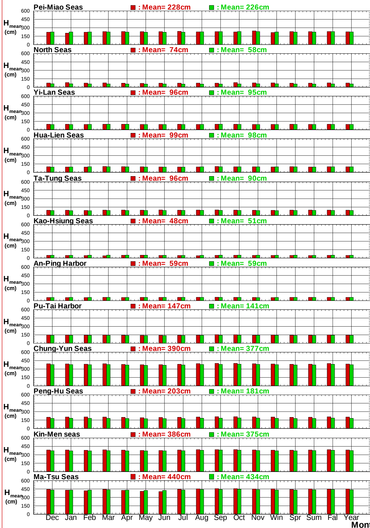
圖7.16 12個港域2018及歷年主要測站每月 (季) 平均潮差比較圖
