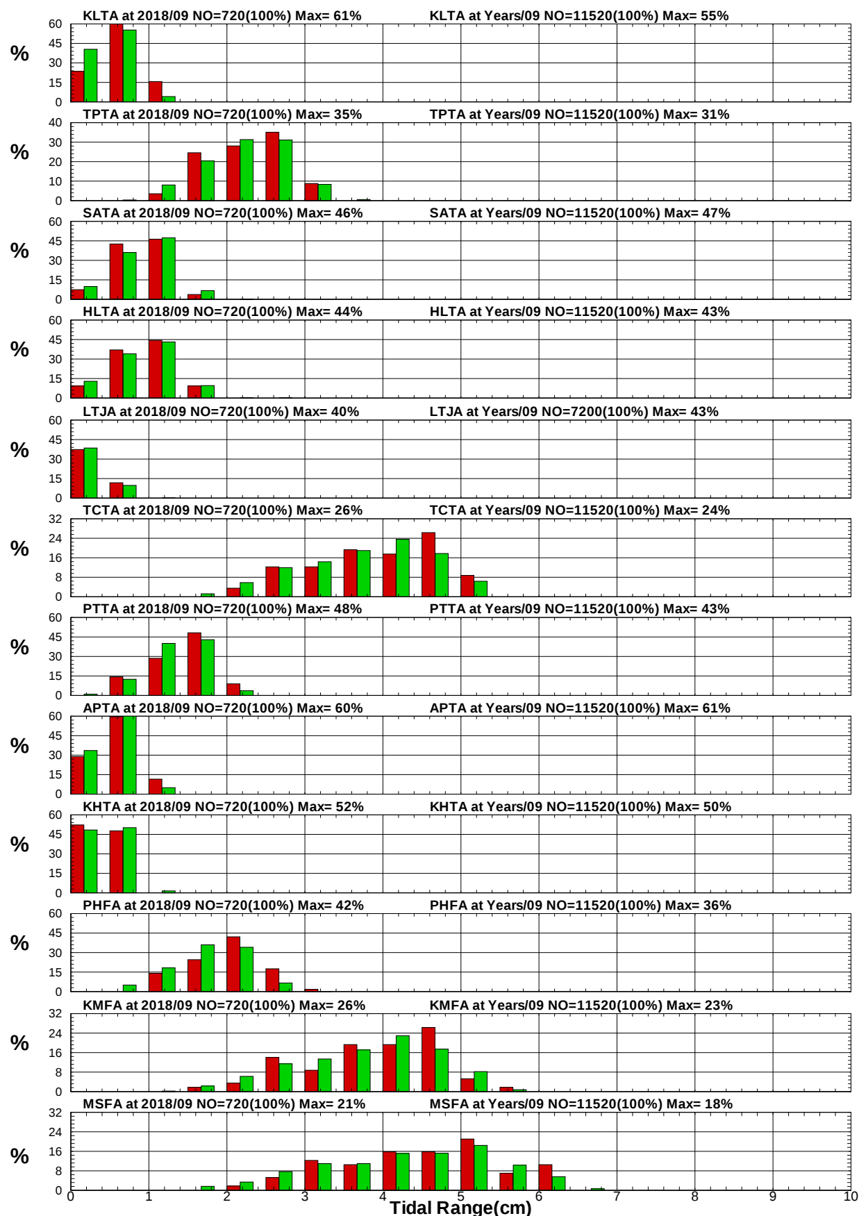
圖8.29 12港域2018年及歷年 9 月潮差統計方塊圖
