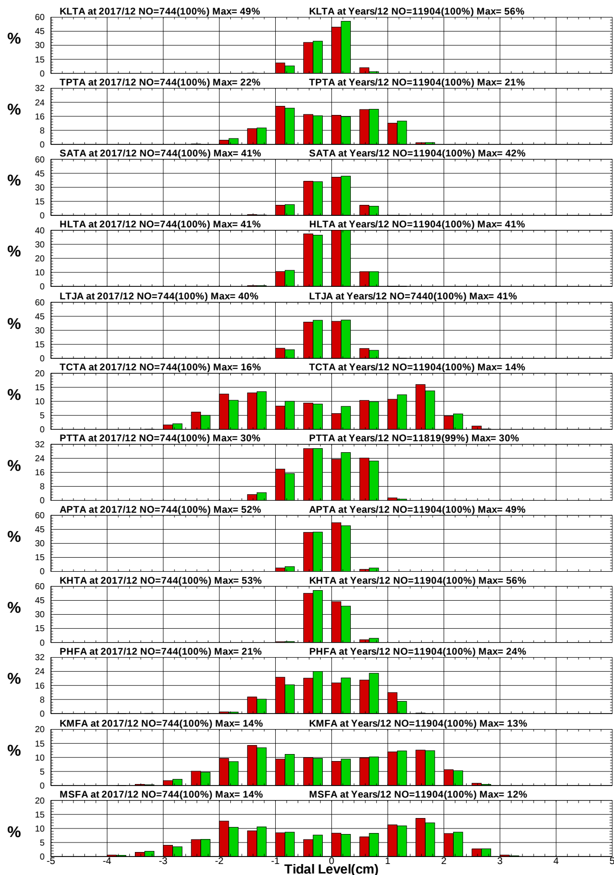
圖8.1 12港域2017年及歷年12月潮位統計方塊圖
