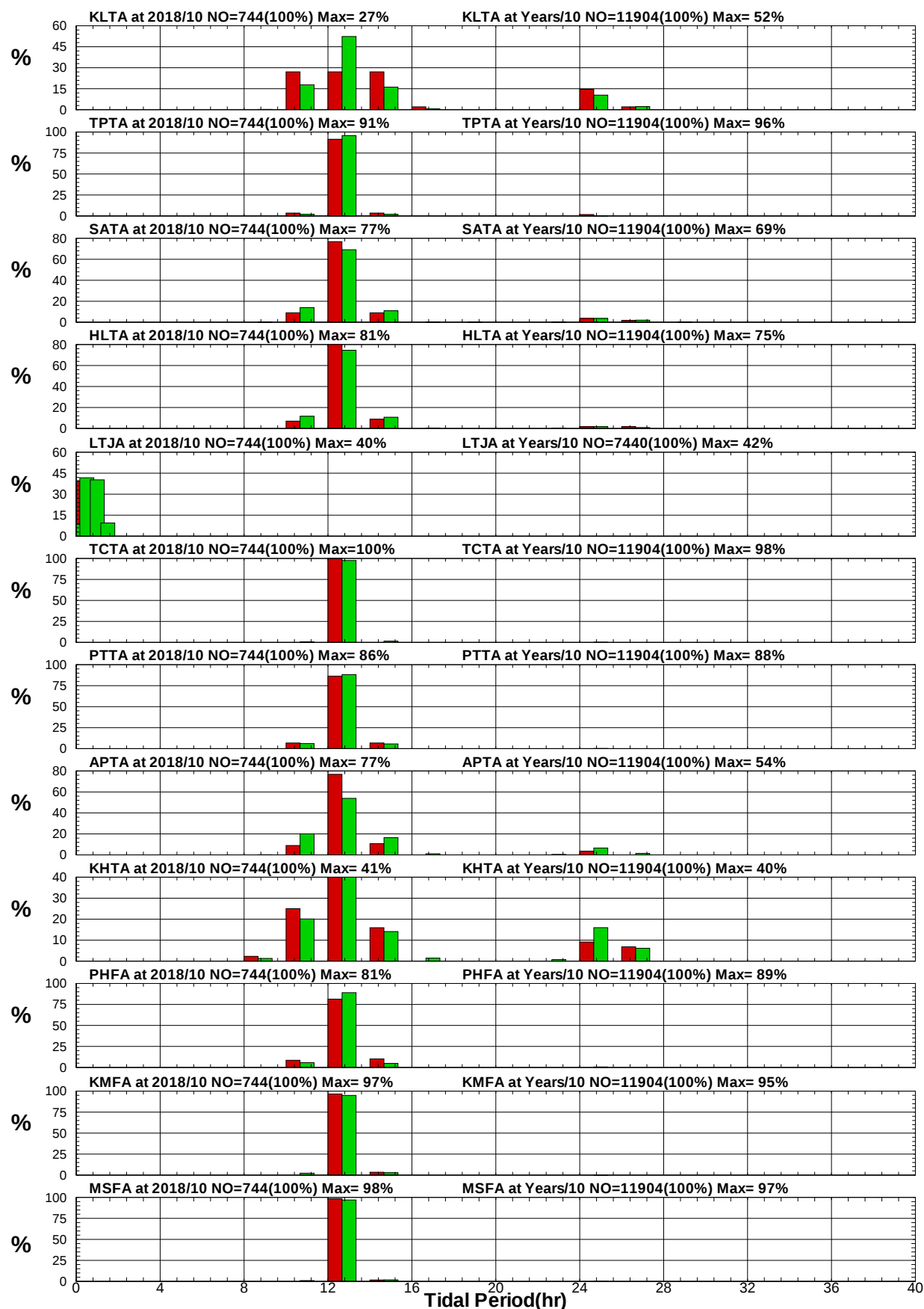
圖8.33 12港域2018年及歷年10月週期統計方塊圖
