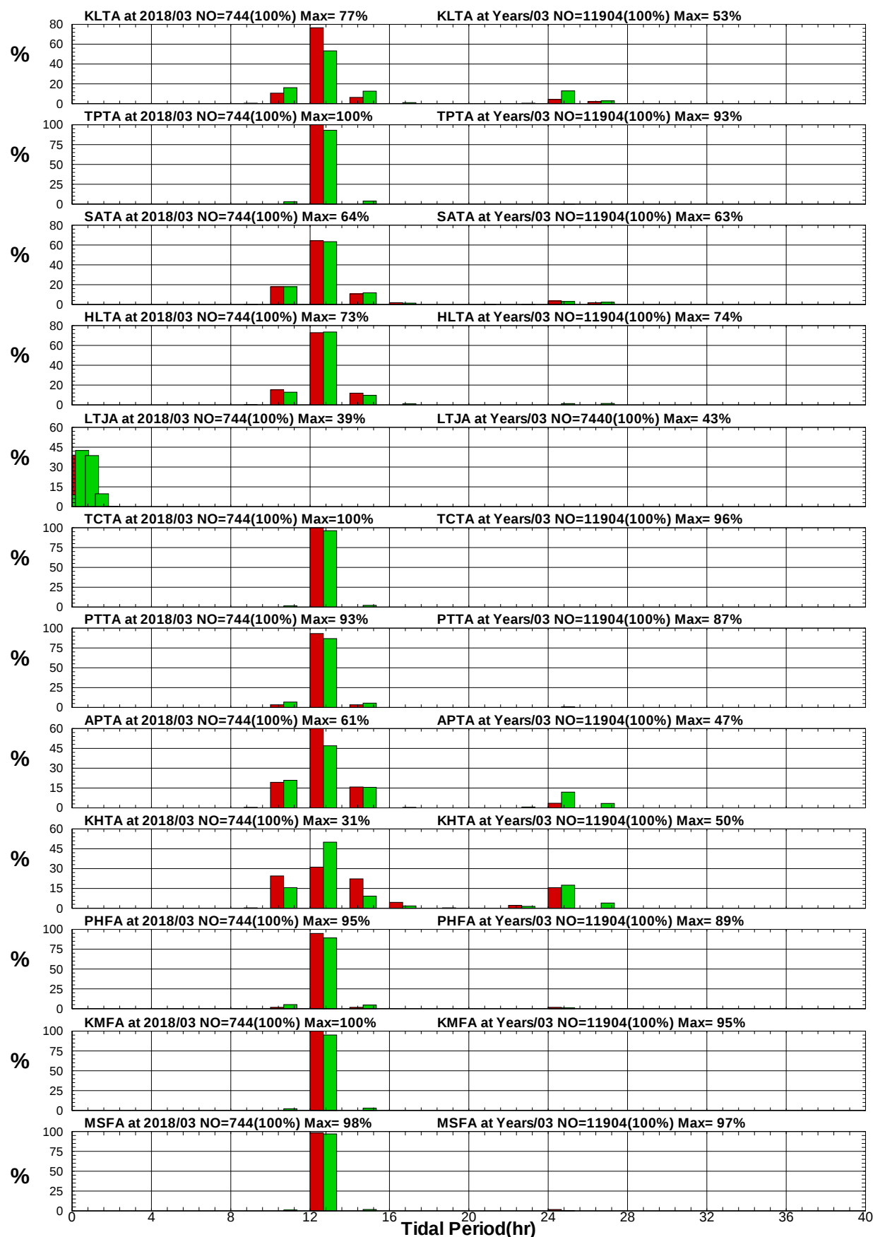
圖8.12 12港域2018年及歷年3月週期統計方塊圖
