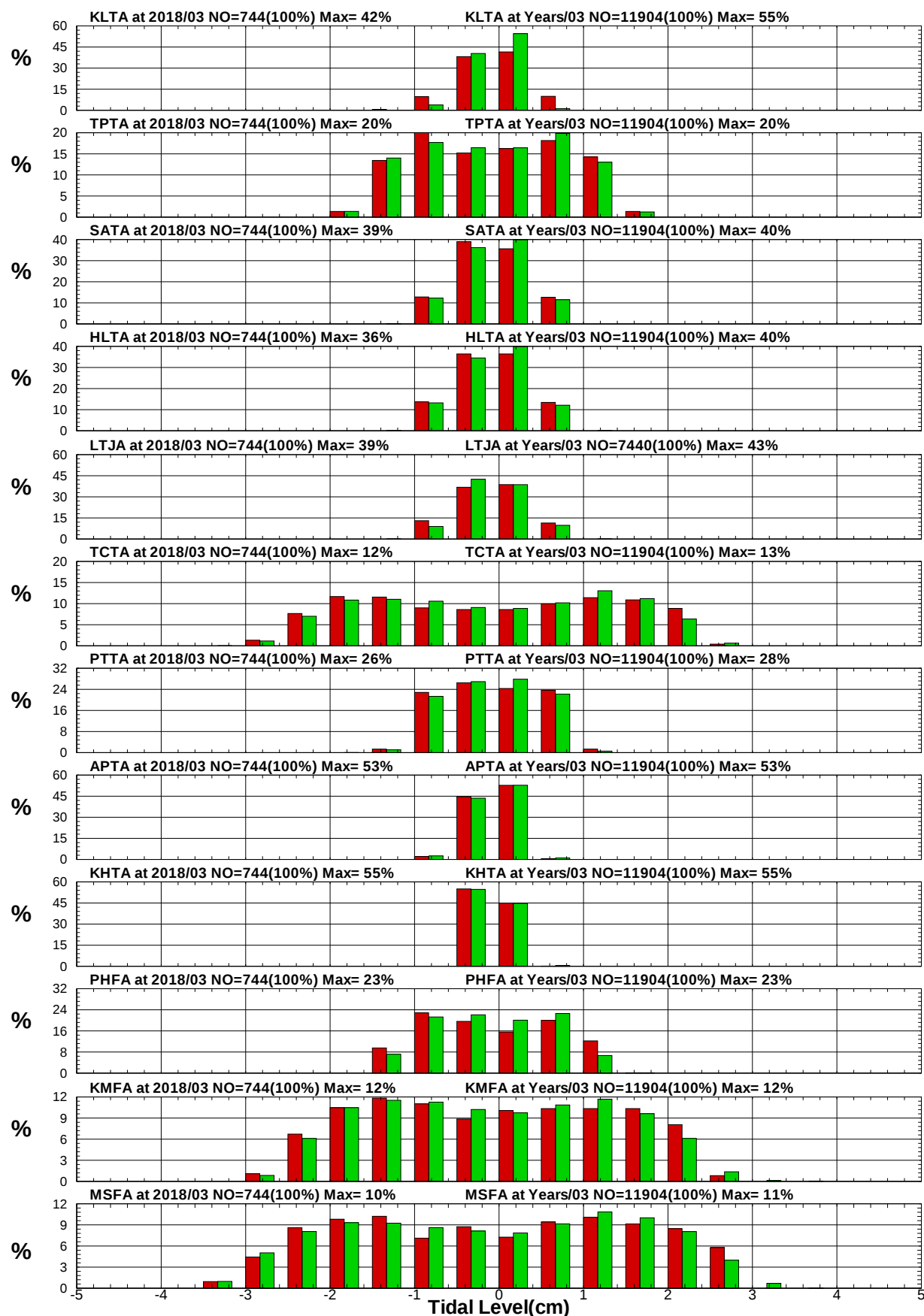
圖8.10 12港域2018年及歷年 3 月潮位統計方塊圖
