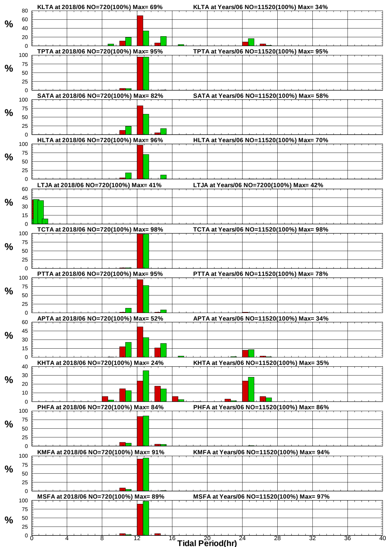
圖8.21 12港域2018年及歷年 6月週期統計方塊圖
