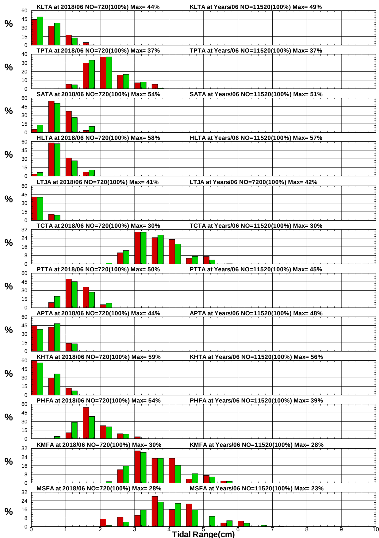
圖8.20 12港域2018年及歷年 6 月潮差統計方塊圖
