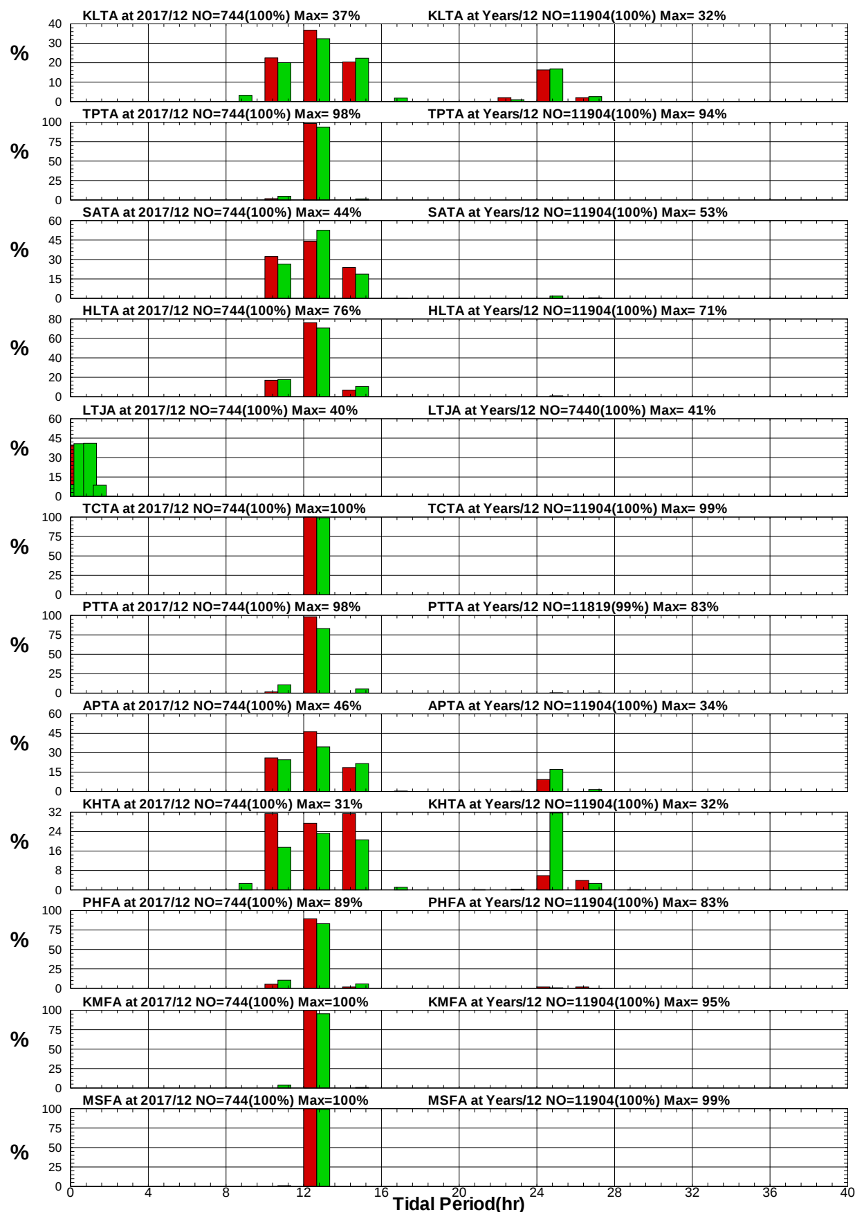
圖8.3 12港域2017年及歷年12月週期統計方塊圖
