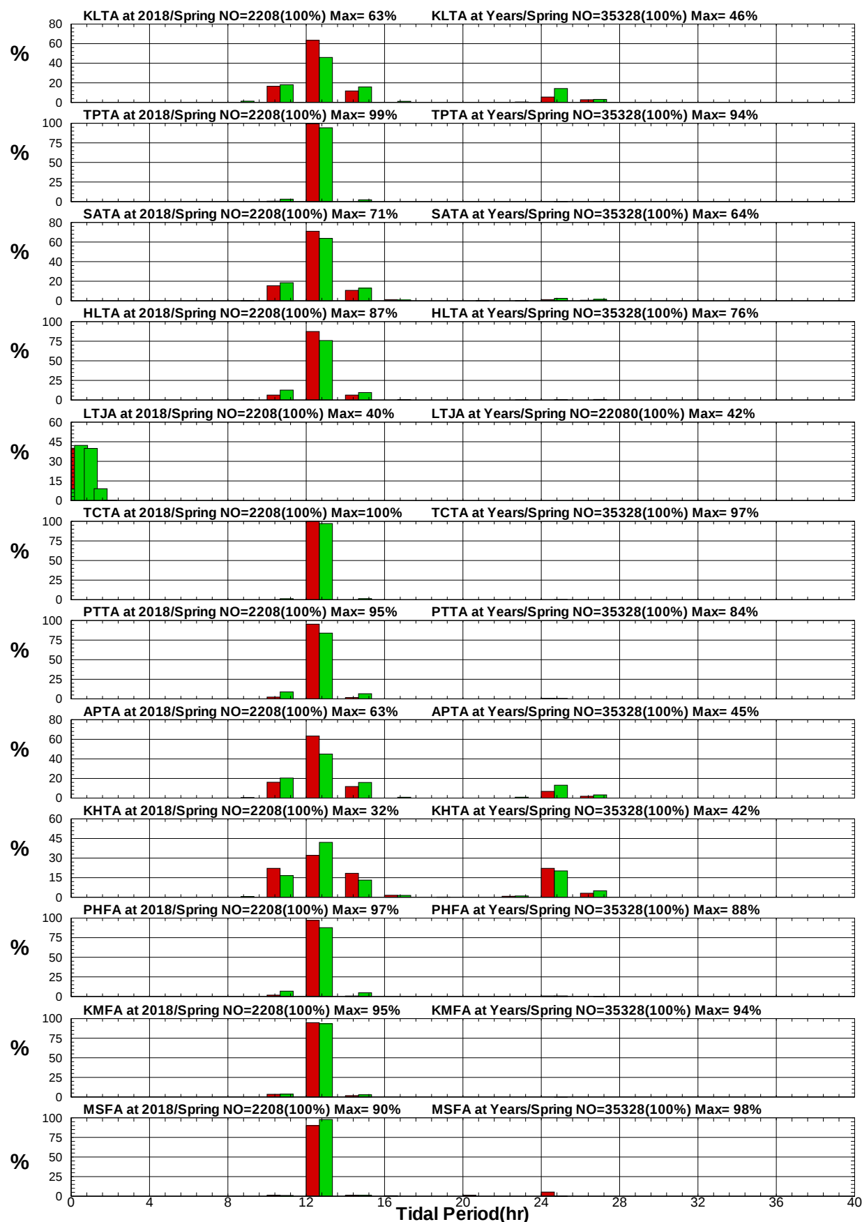
圖8.42 12港域2018年及歷年春季週期統計方塊圖
