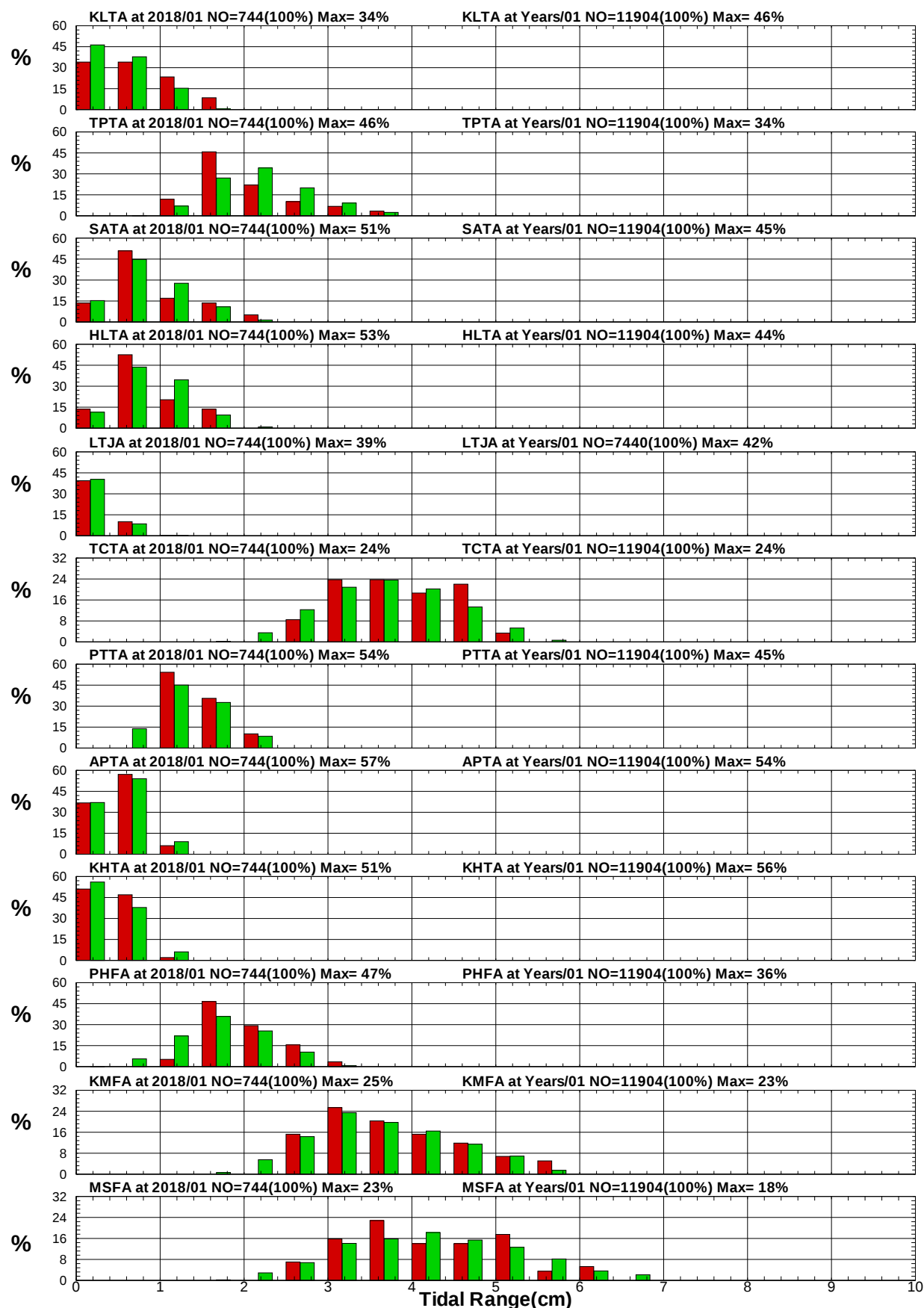
圖8.5 12港域2018年及歷年 1 月潮差統計方塊圖
