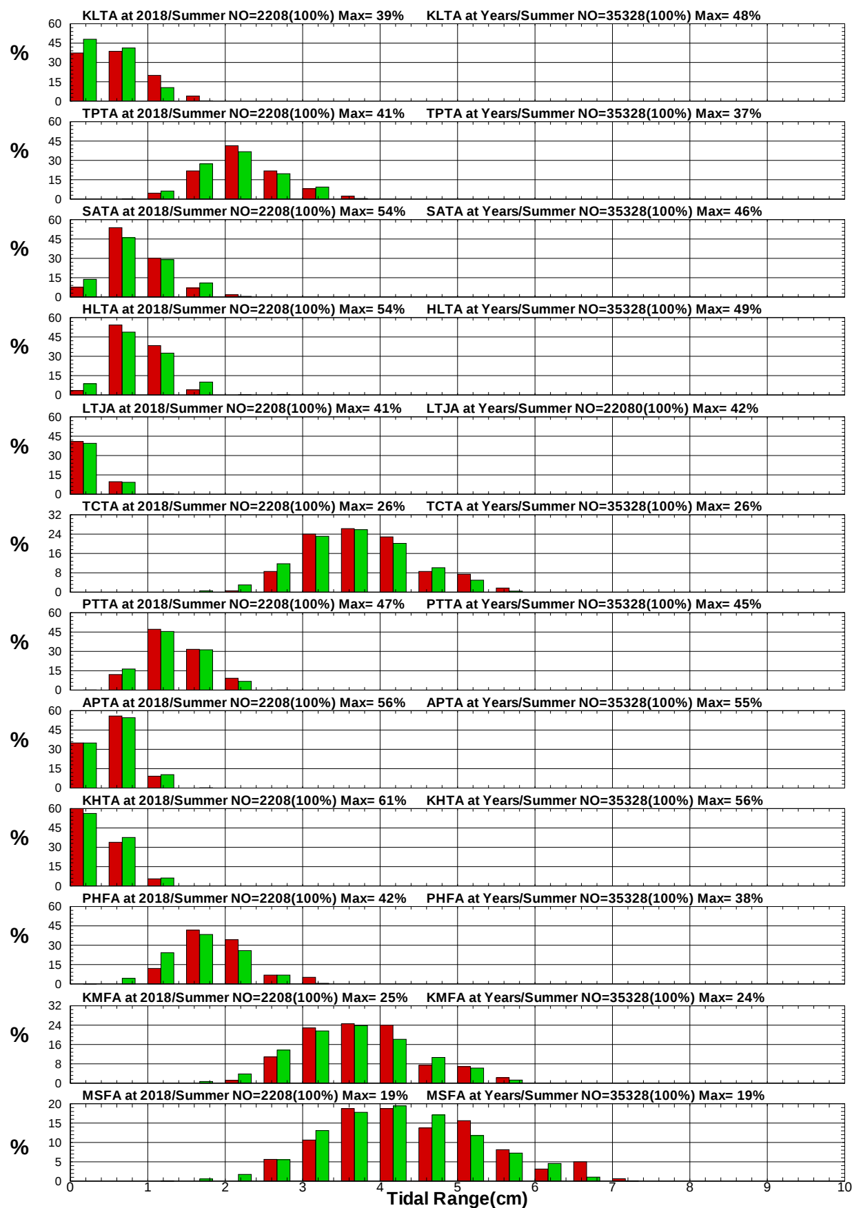
圖8.44 12港域2018年及歷年夏季潮差統計方塊圖
