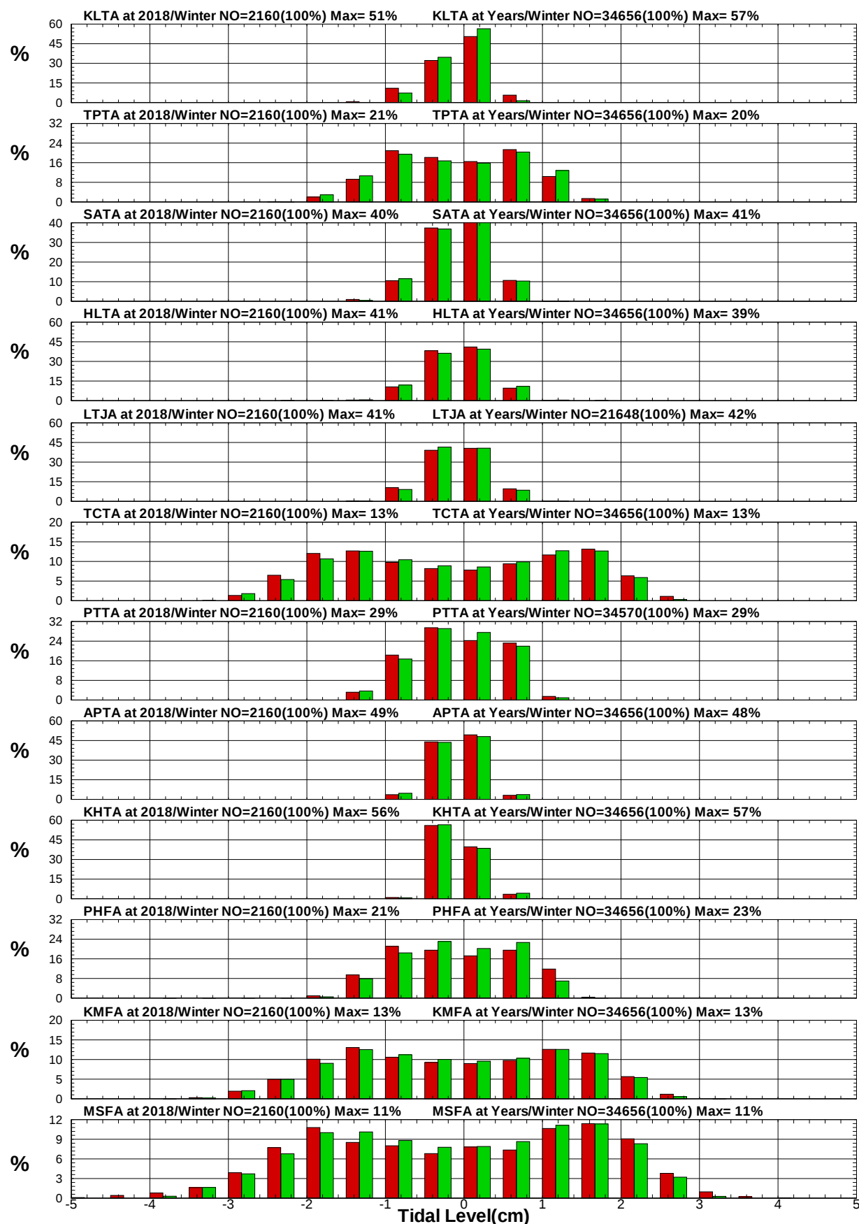
圖8.37 12港域2018年及歷年冬季潮位統計方塊圖
