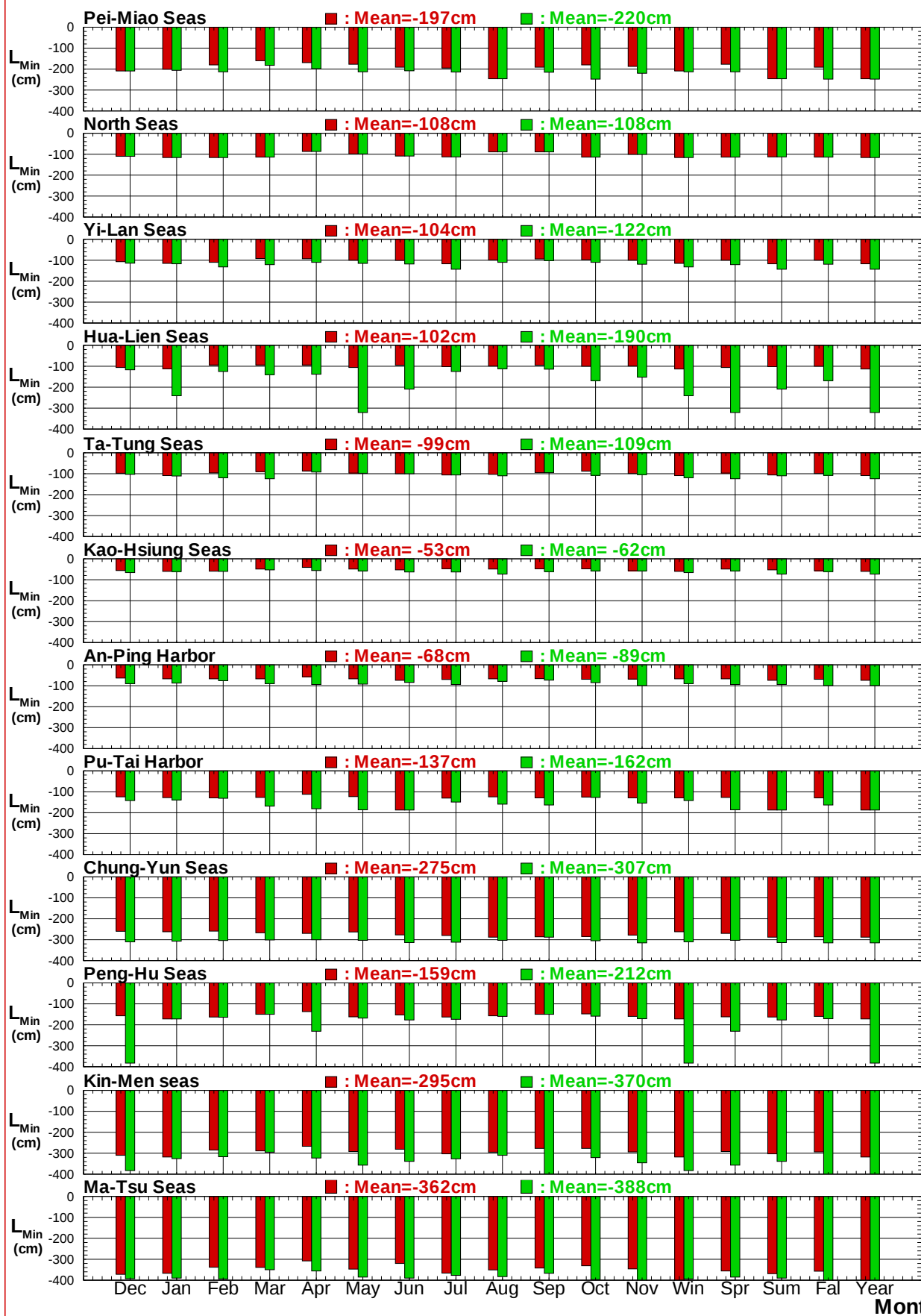
圖7.13 12個港域2018及歷年主要測站每月 (季) 最低潮位比較圖
