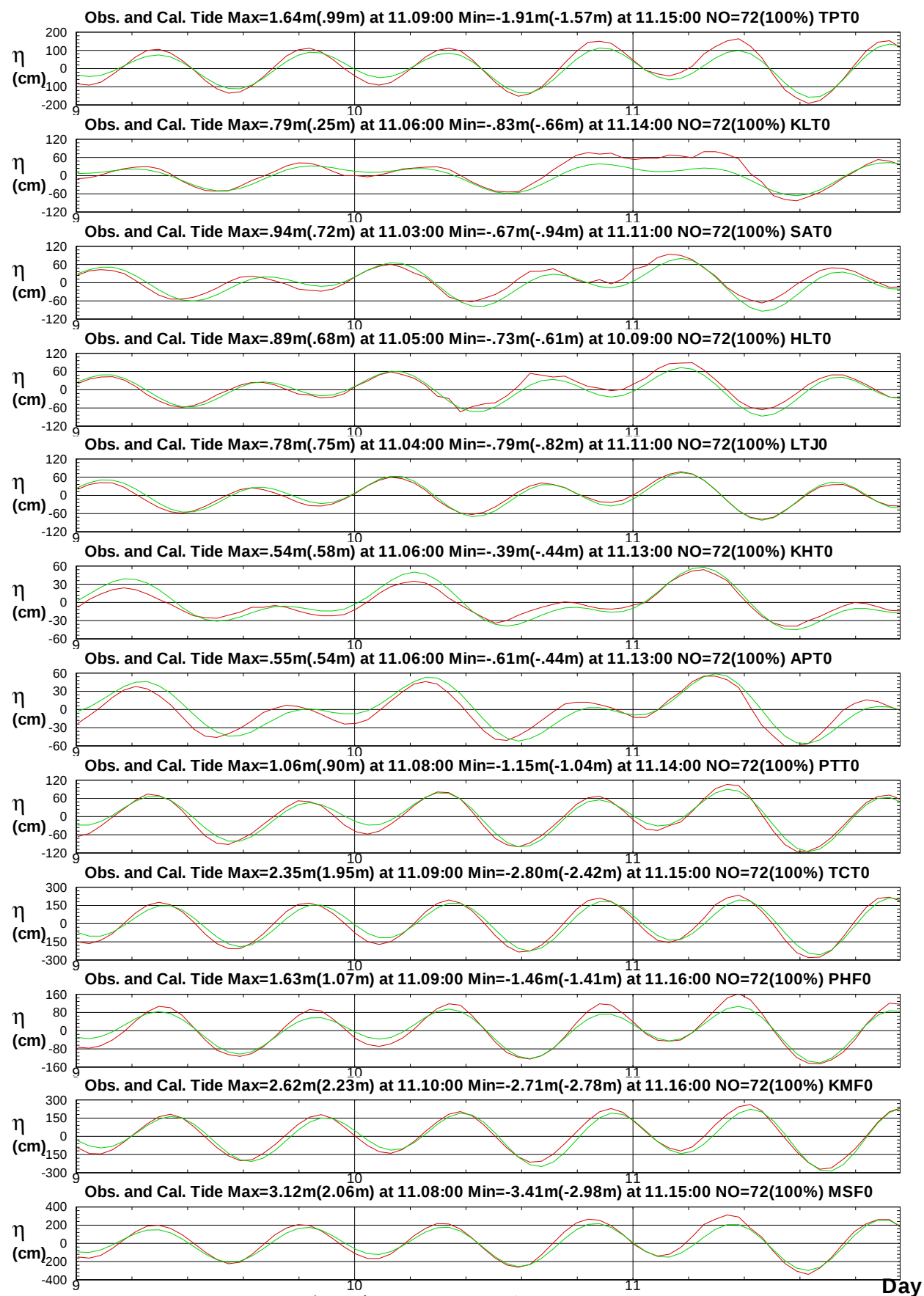
圖9.1 2018年瑪莉亞颱風12海域觀測潮位歷線圖 (細: 天文潮)
