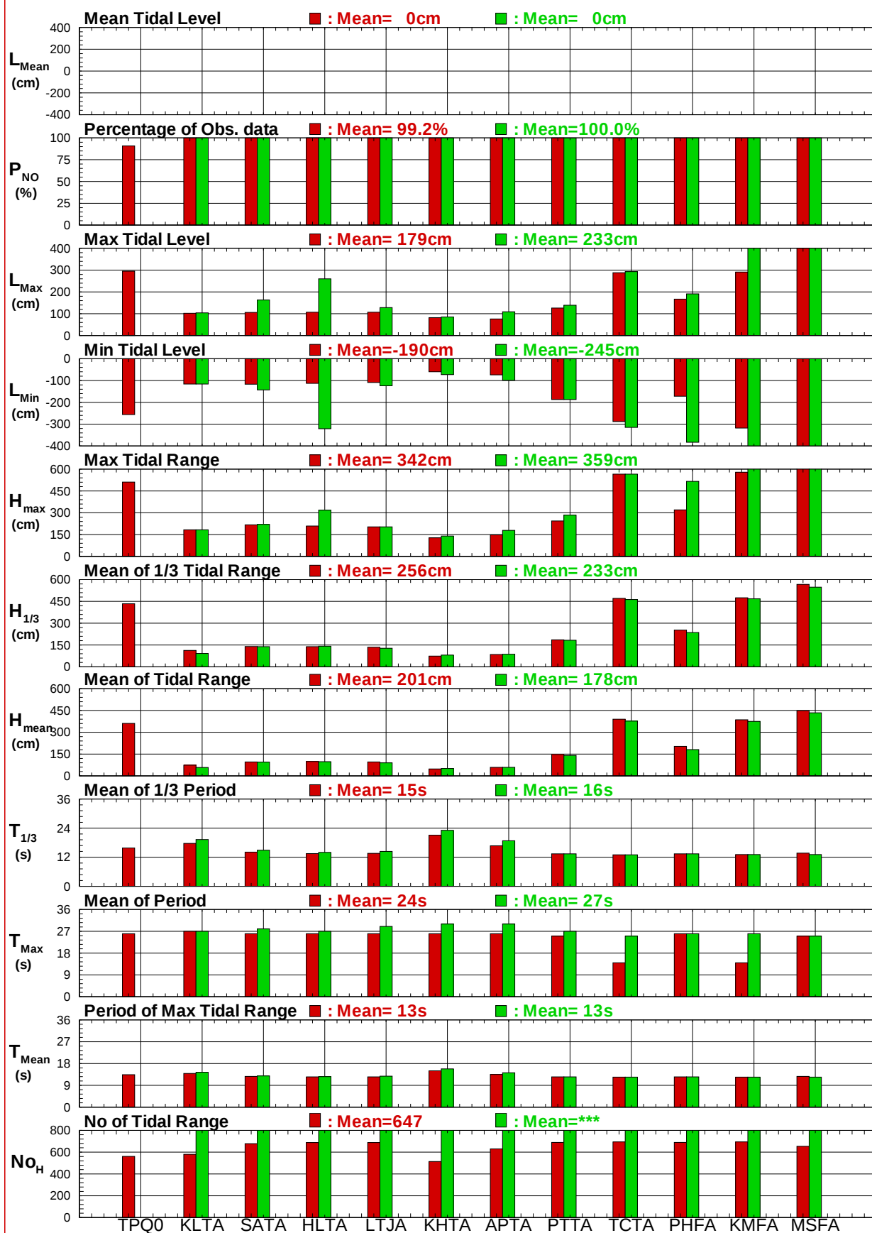
圖7.5 12個港域2018及歷年主要測站整年潮位比較圖
