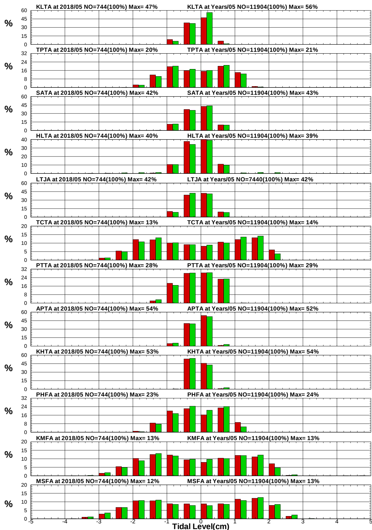
圖8.16 12港域2018年及歷年 5月潮位統計方塊圖
