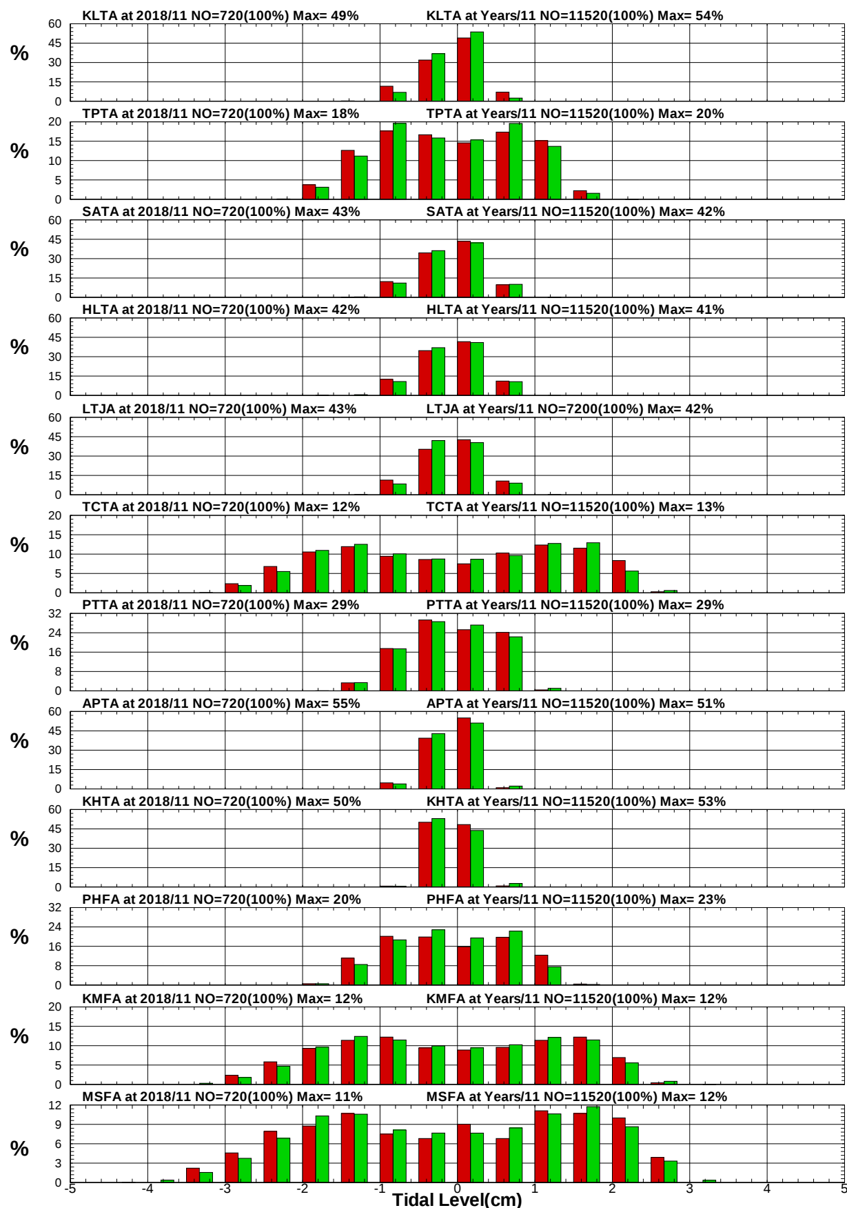
圖8.34 12港域2018年及歷年11月潮位統計方塊圖
