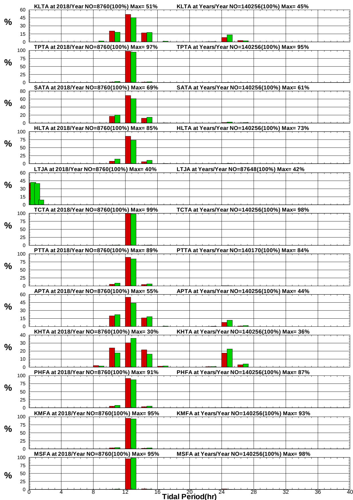
圖8.51 12港域2018年及歷年整年週期統計方塊圖
