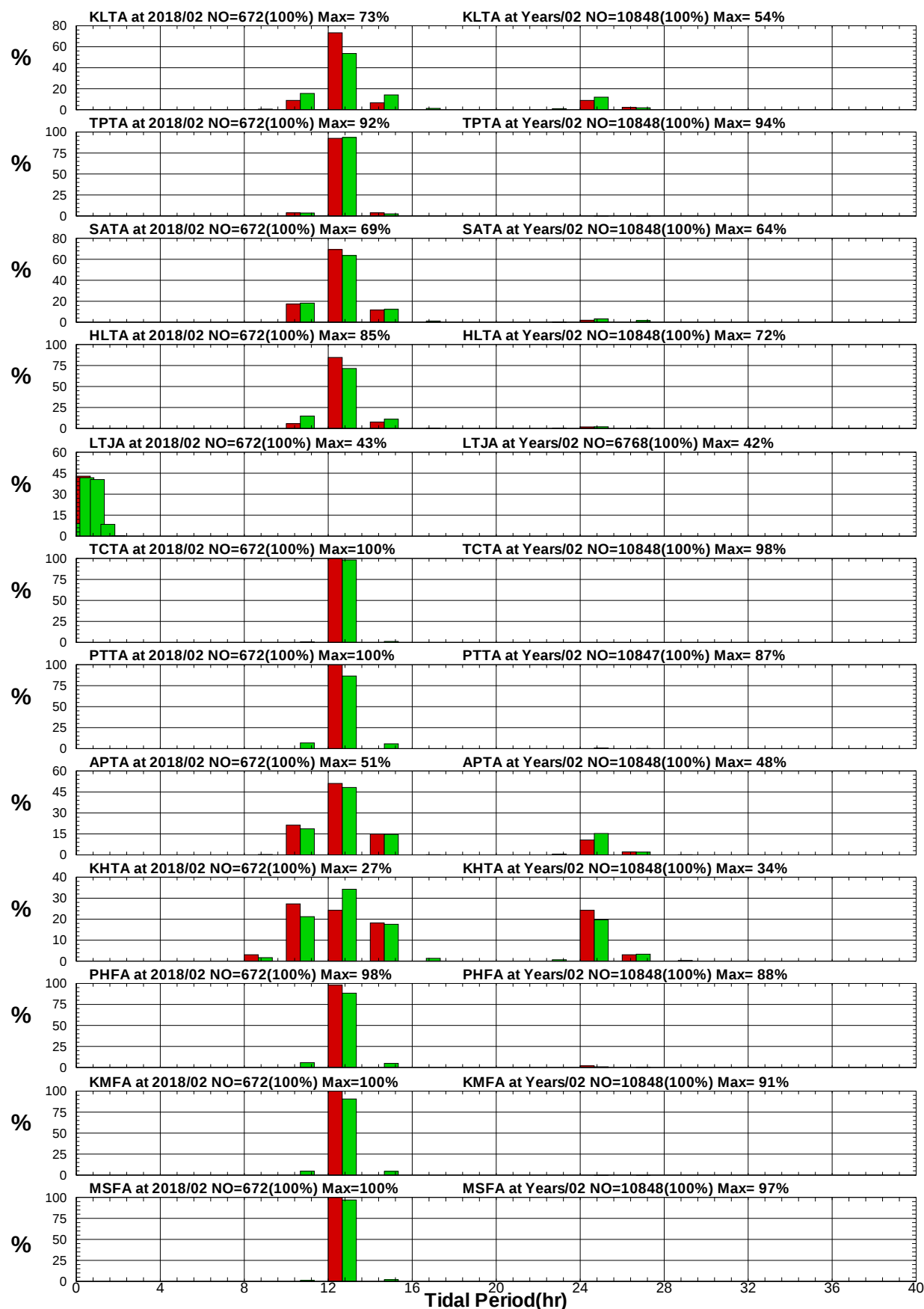
圖8.9 12港域2018年及歷年 2月週期統計方塊圖
