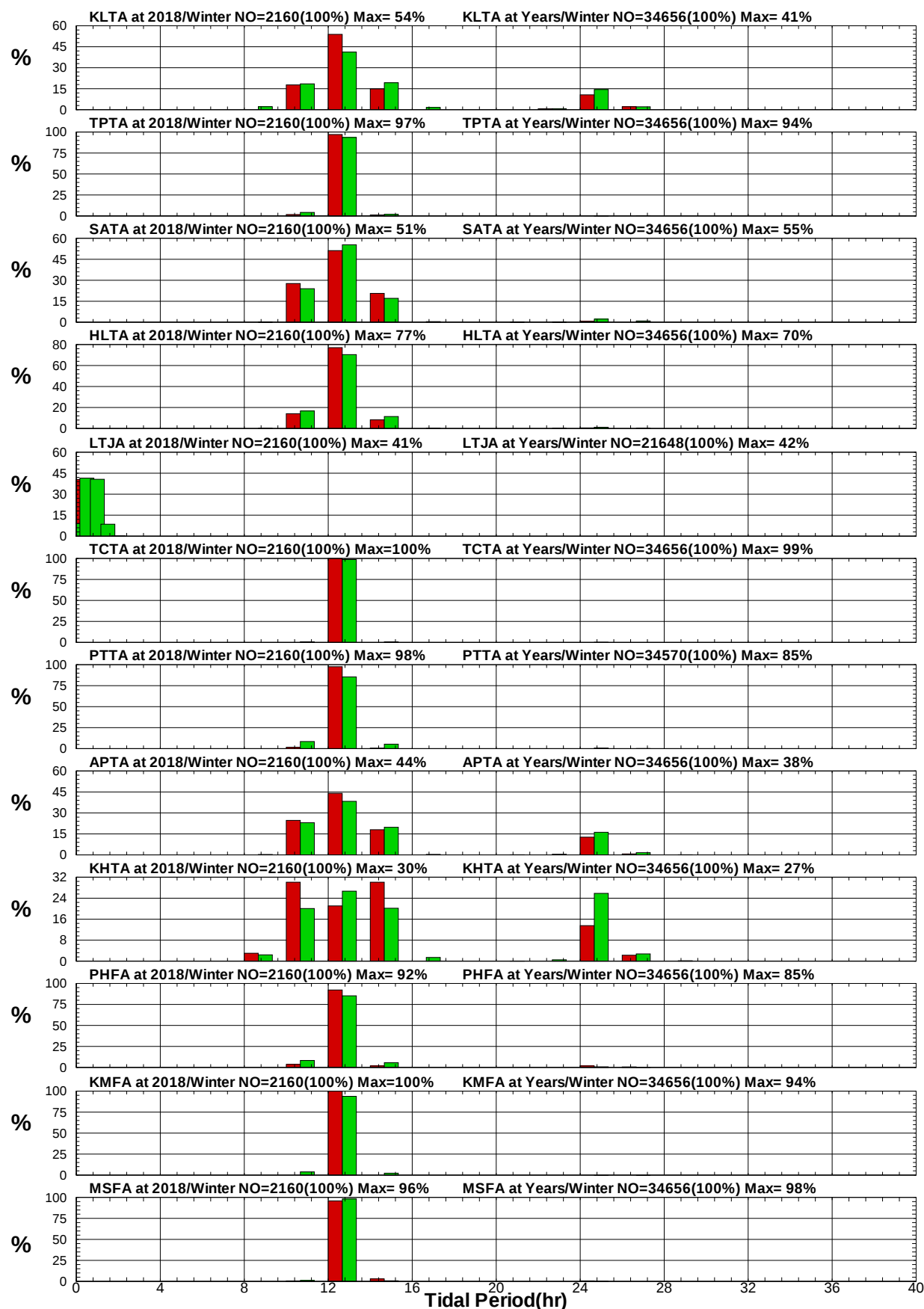
圖8.39 12港域2018年及歷年冬季週期統計方塊圖
