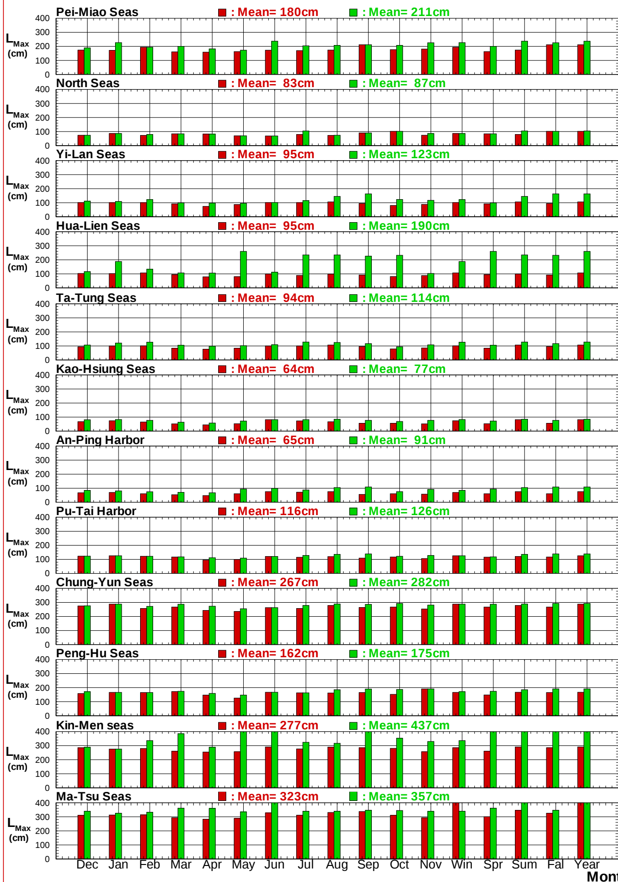
圖7.12 12個港域2018及歷年主要測站每月 (季) 最高潮位比較圖
