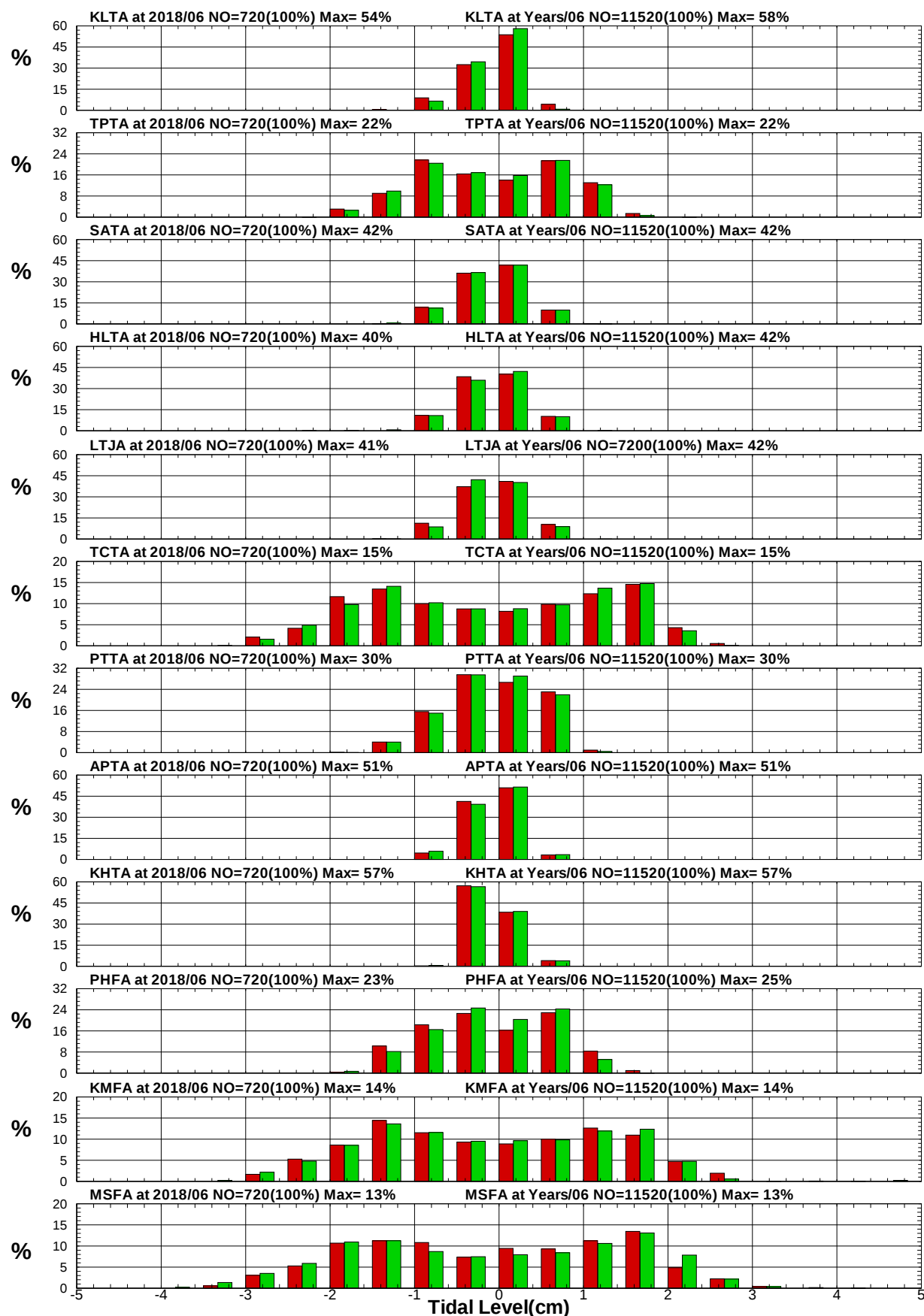
圖8.19 12港域2018年及歷年 6 月潮位統計方塊圖
