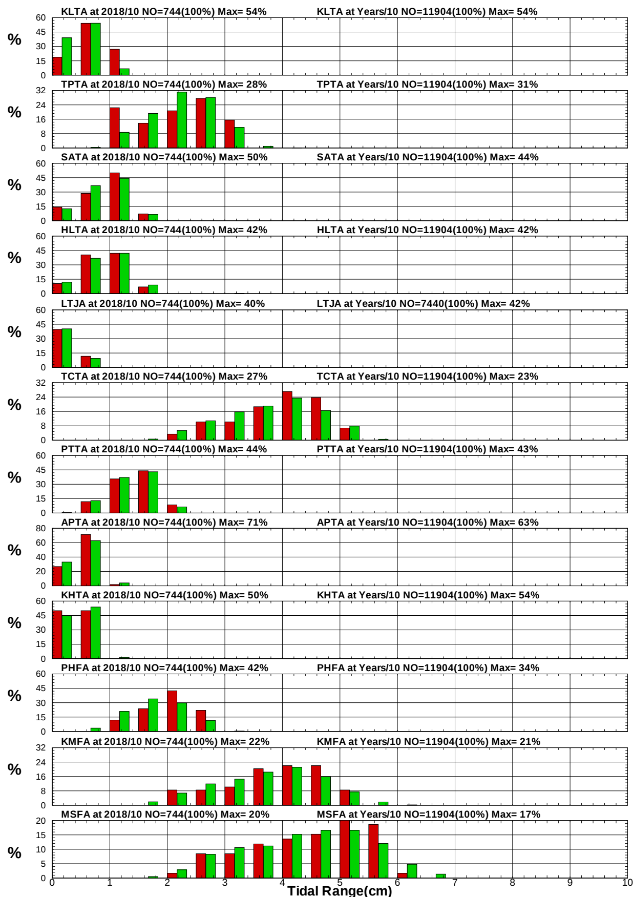
圖8.32 12港域2018年及歷年10月潮差統計方塊圖
