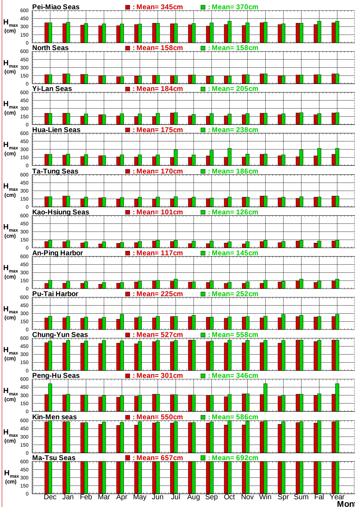
圖7.14 12個港域2018及歷年主要測站每月 (季) 最大潮差比較圖
