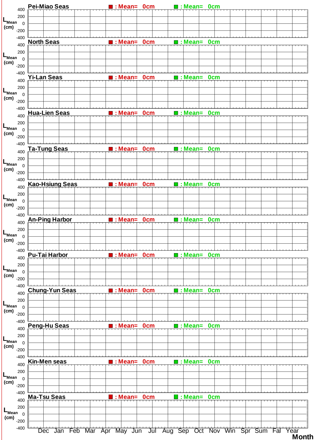
圖7.10 12個港域2018及歷年主要測站每月(季)平均潮位比較圖
