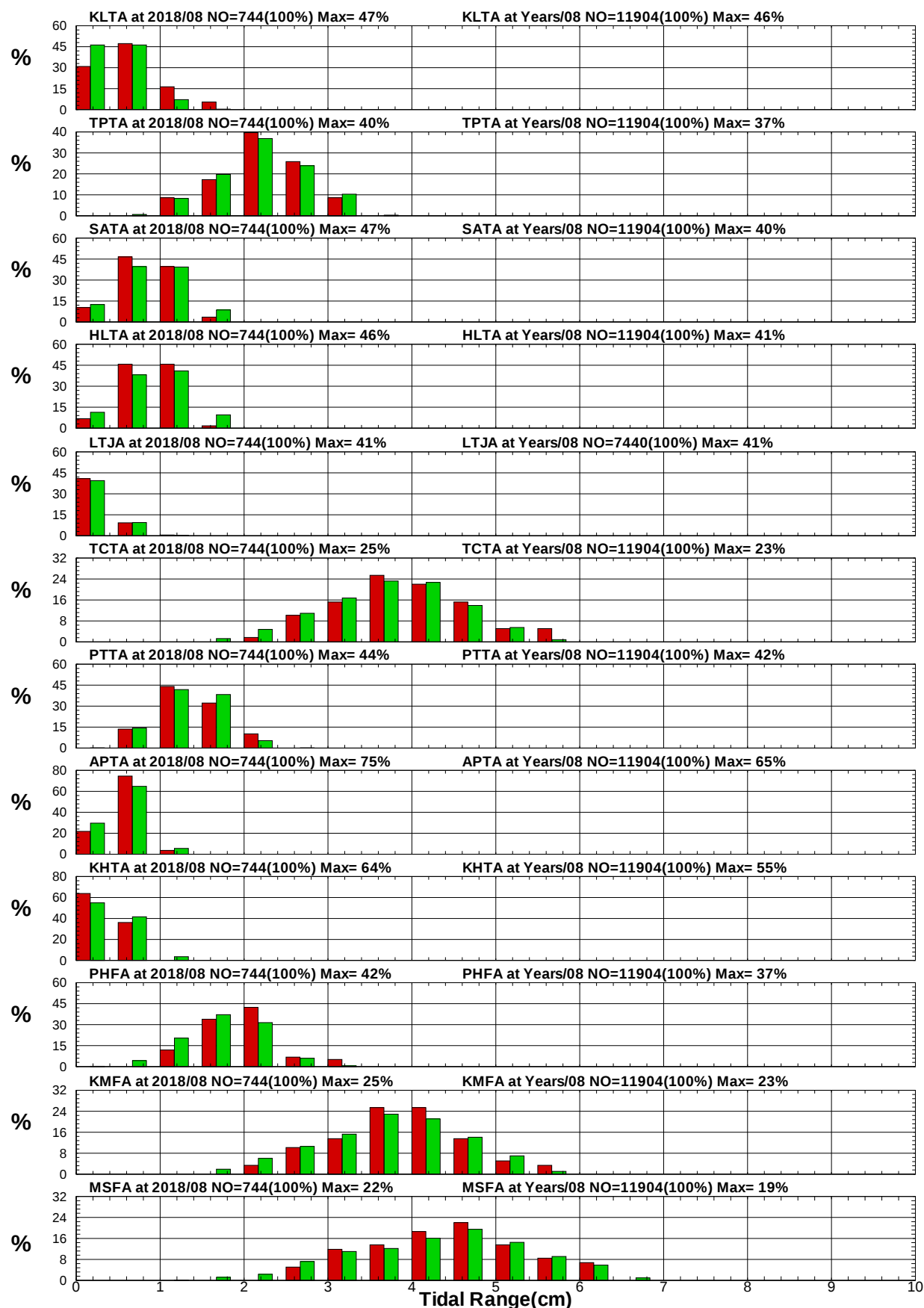
圖8.26 12港域2018年及歷年 8 月潮差統計方塊圖
