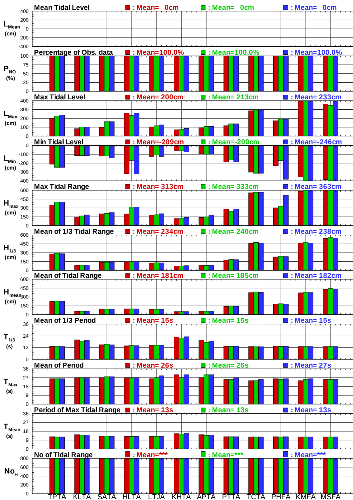
圖7.9 12個港域歷年主要測站春、秋及整年潮位比較圖
