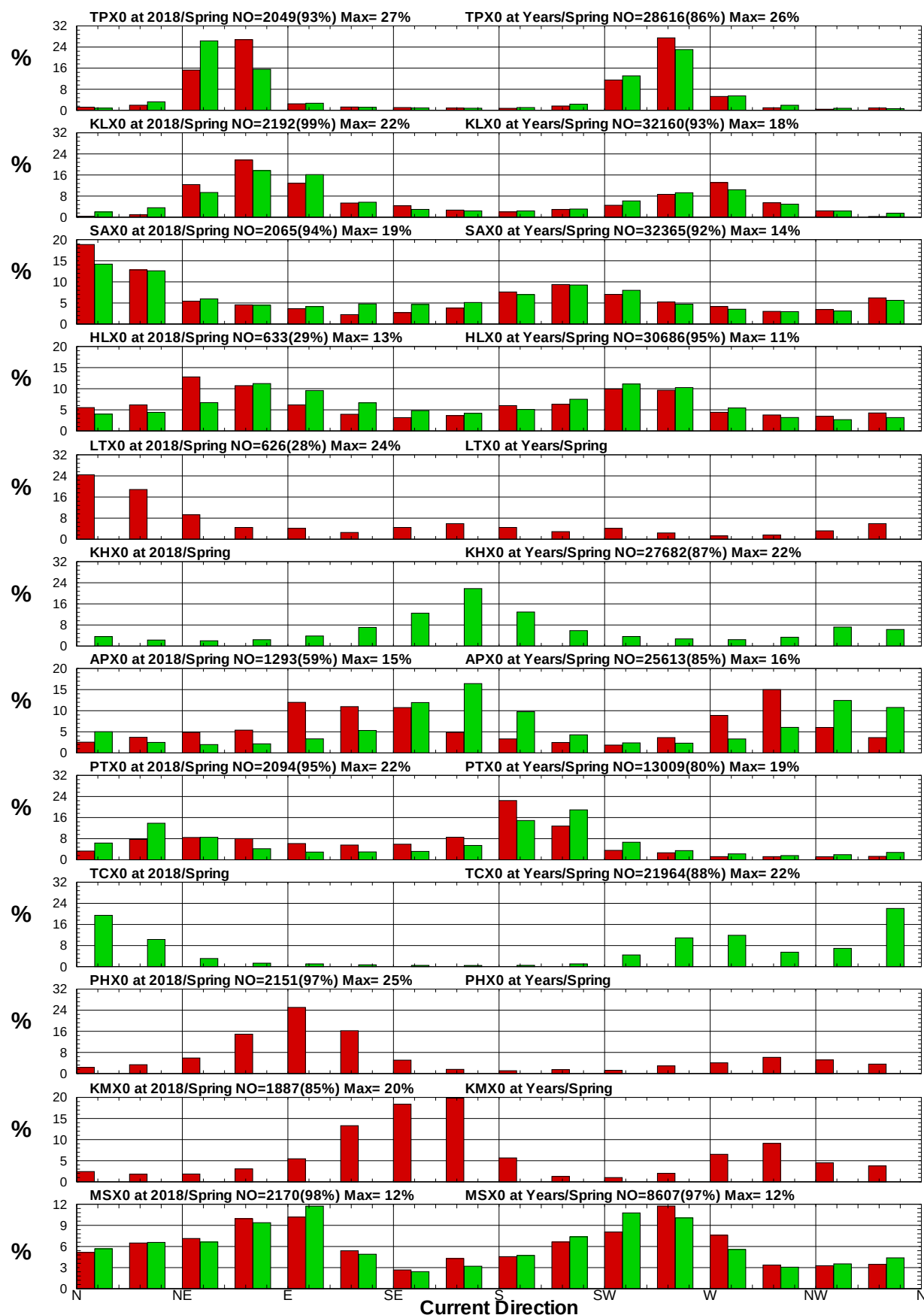
圖8.28 12港域2018年及歷年春季流向統計方塊圖
