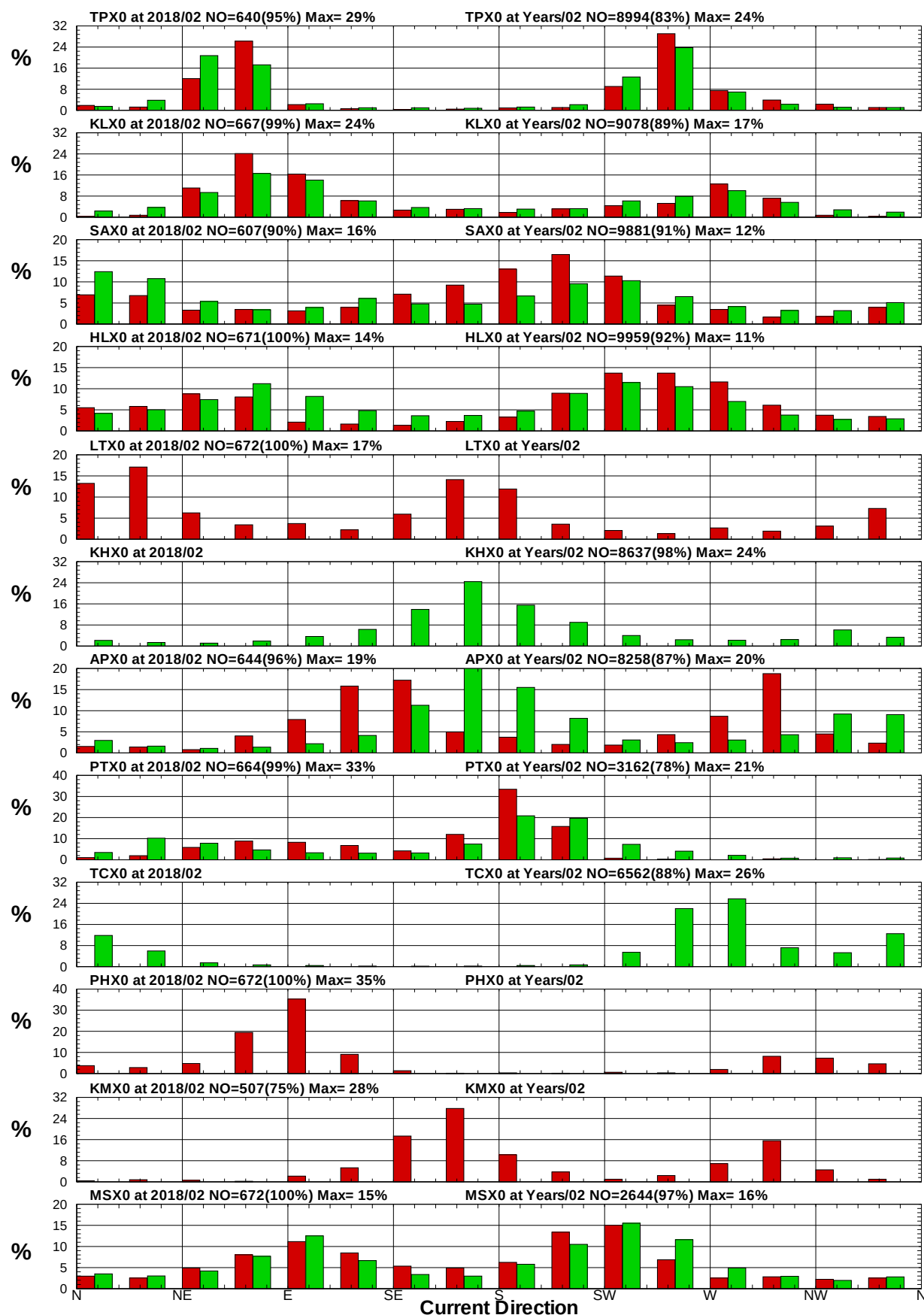
圖8.6 12港域2018年及歷年 2月流向統計方塊圖
