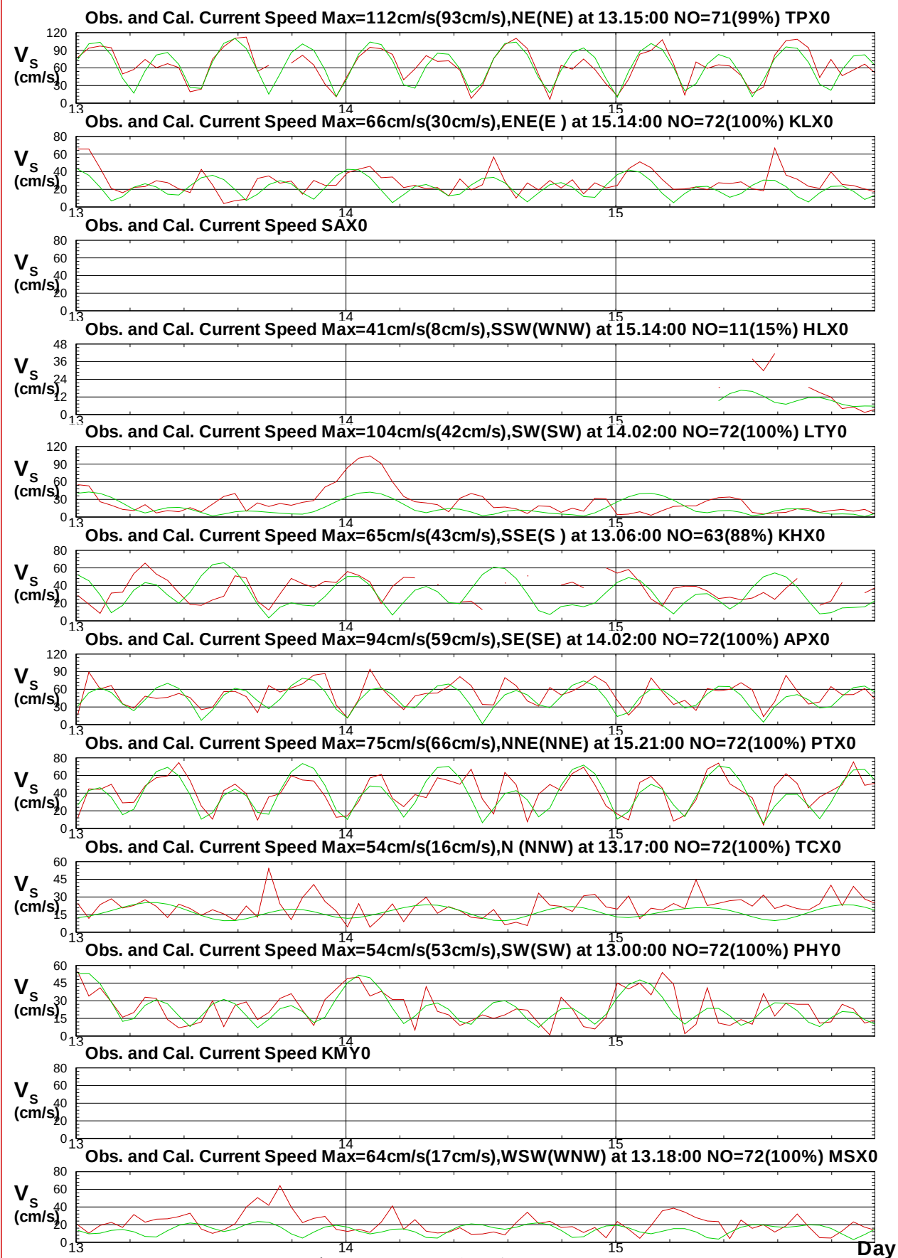
圖10.3 2018年山竹 颱風12海域觀測流速歷線圖 (綠色: 潮流)
