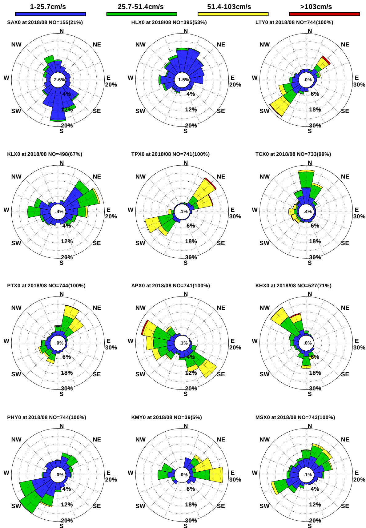
圖9.17 12港域2018年8月觀測海流玫瑰比較圖
