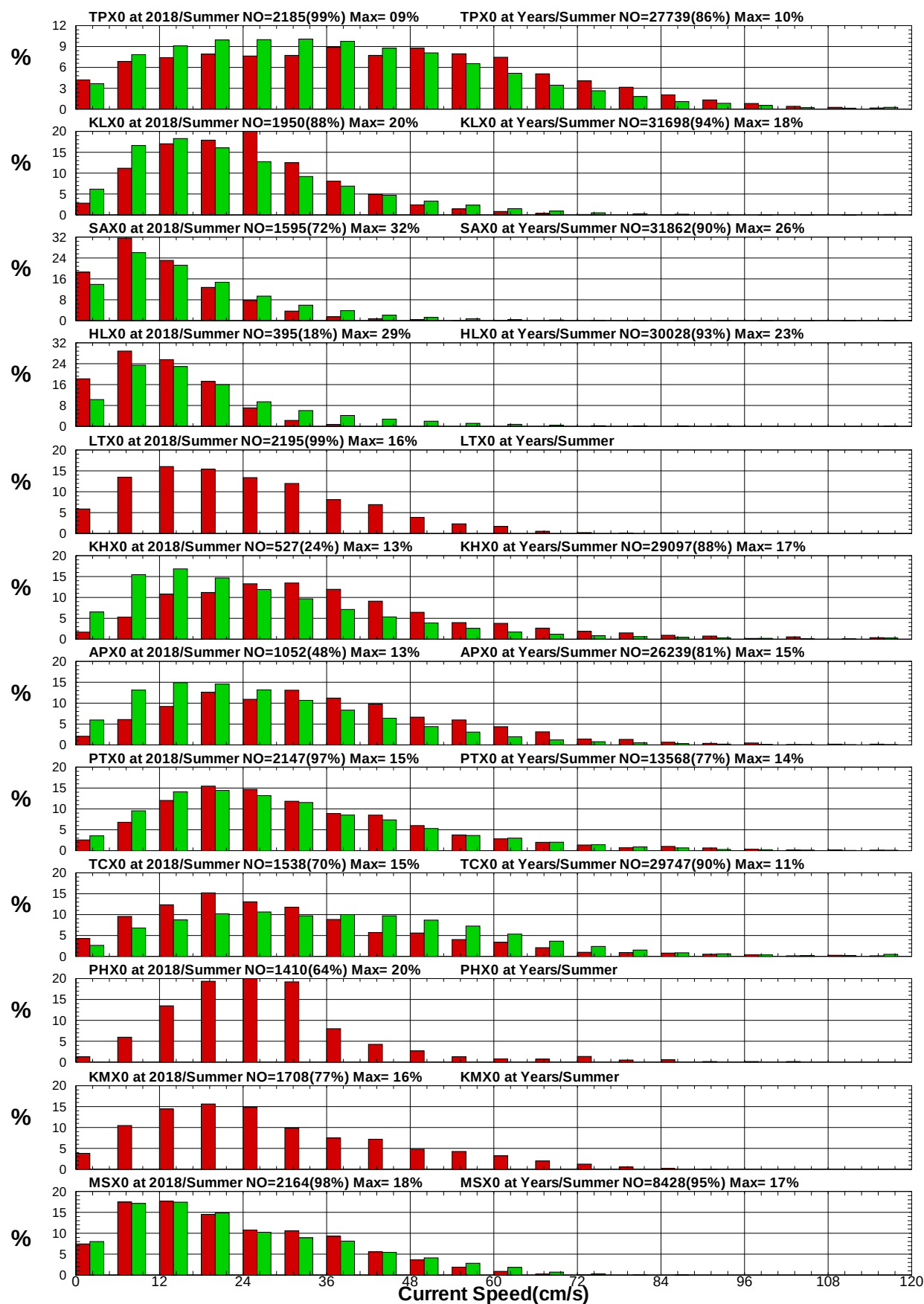
圖8.29 12港域2018年及歷年夏季流速統計方塊圖
