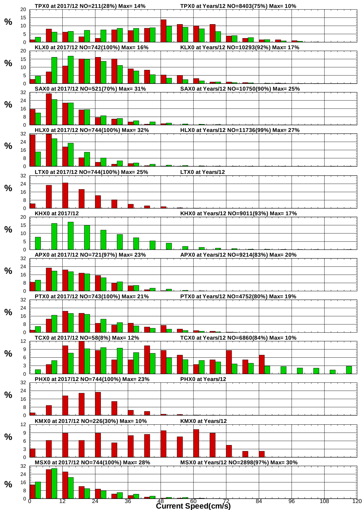
圖8.1 12港域2017年及歷年12月流速統計方塊圖
