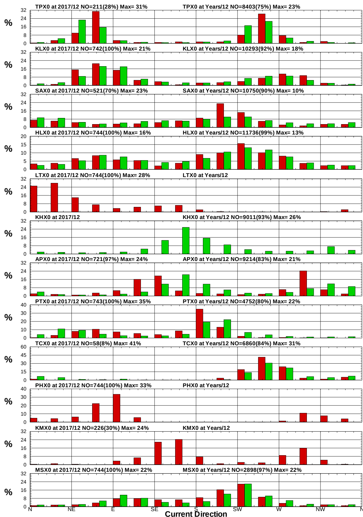
圖8.2 12港域2017年及歷年12月流向統計方塊圖
