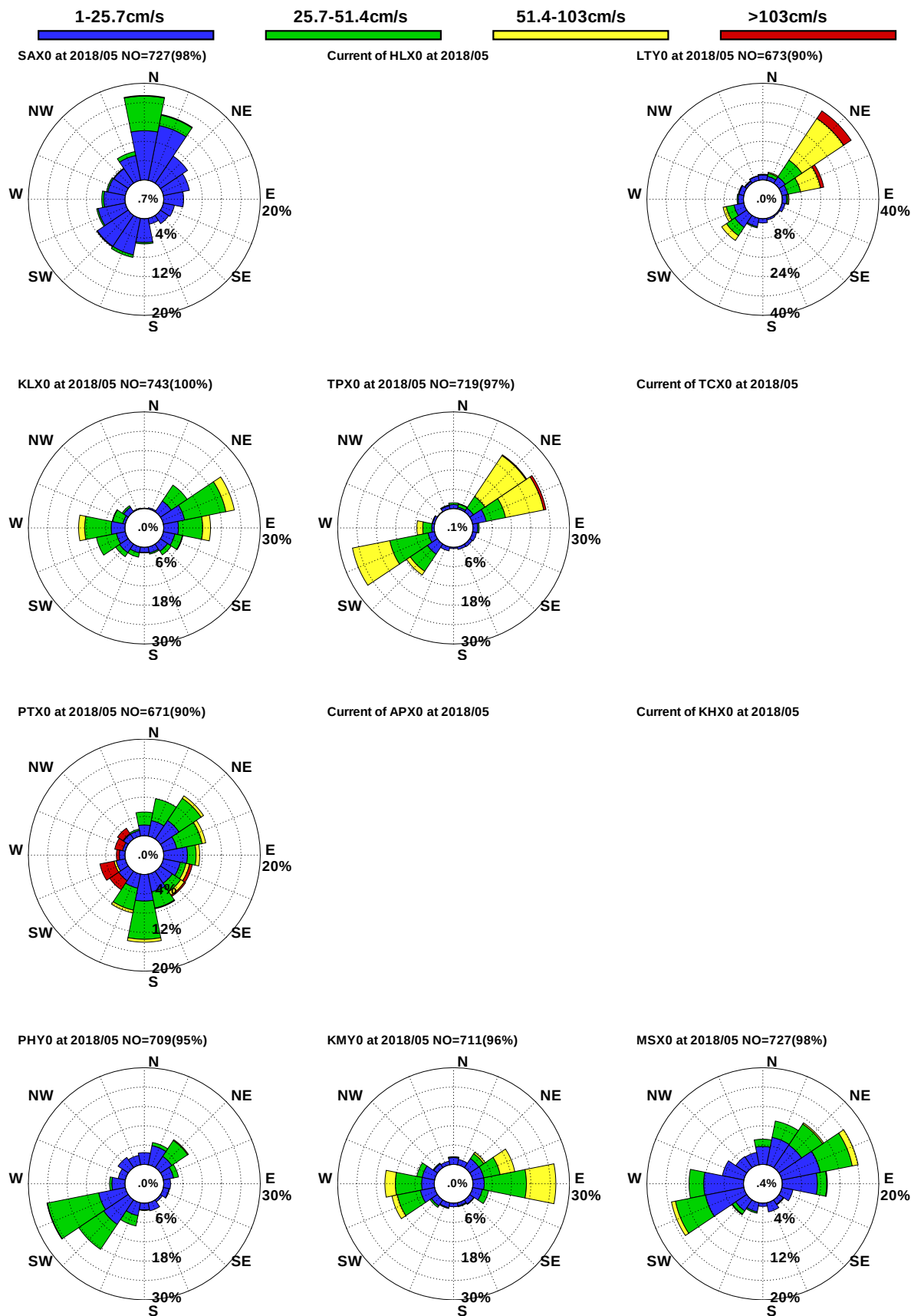
圖9.11 12港域2018年 5月觀測海流玫瑰比較圖
