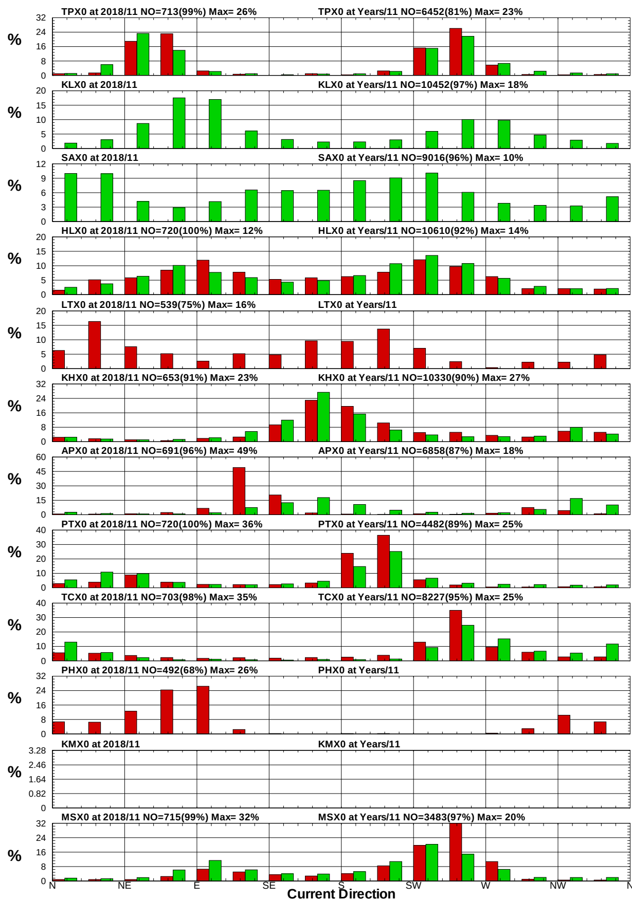
圖8.24 12港域2018年及歷年11月流向統計方塊圖
