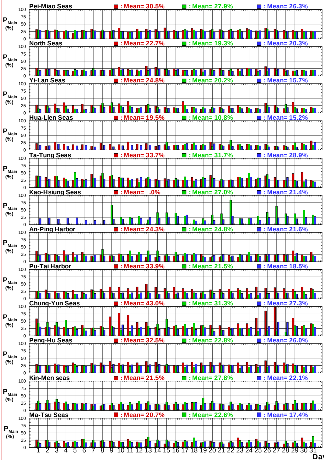
圖7.6f 2018年12港域冬, 夏及整年主要測站每日主要流向百分比圖
