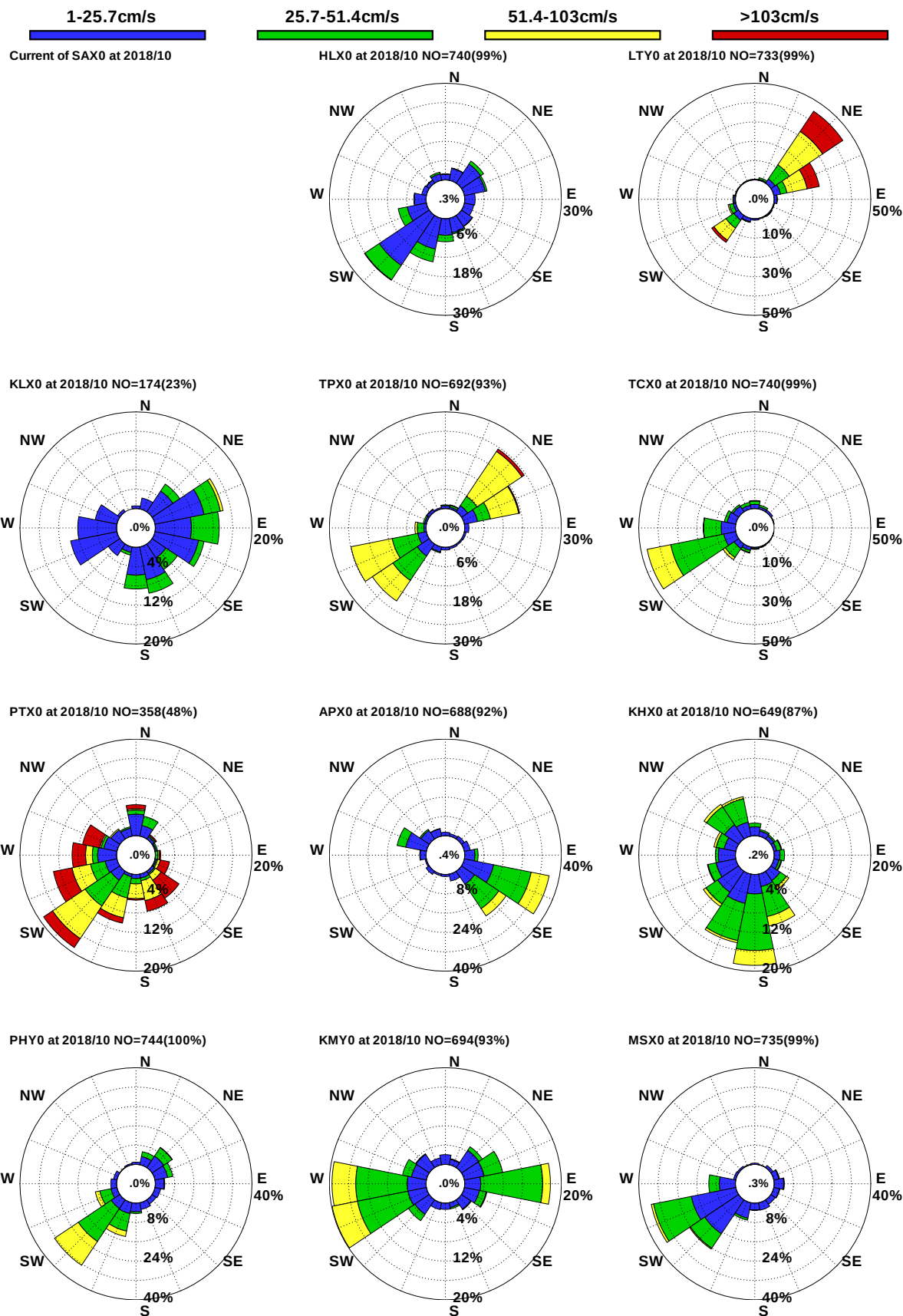
圖9.21 12港域2018年10月觀測海流玫瑰比較圖
