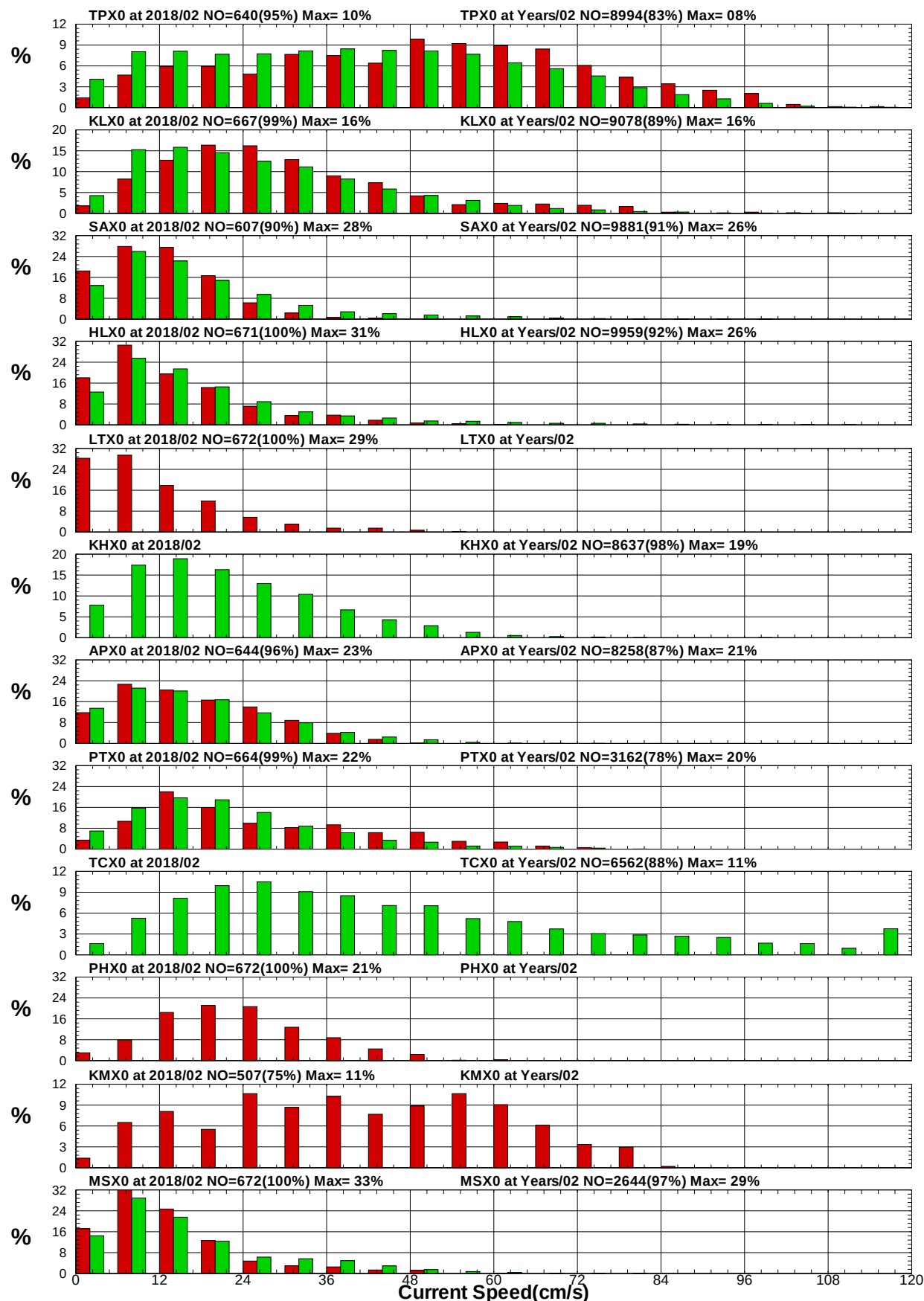
圖8.5 12港域2018年及歷年 2月流速統計方塊圖
