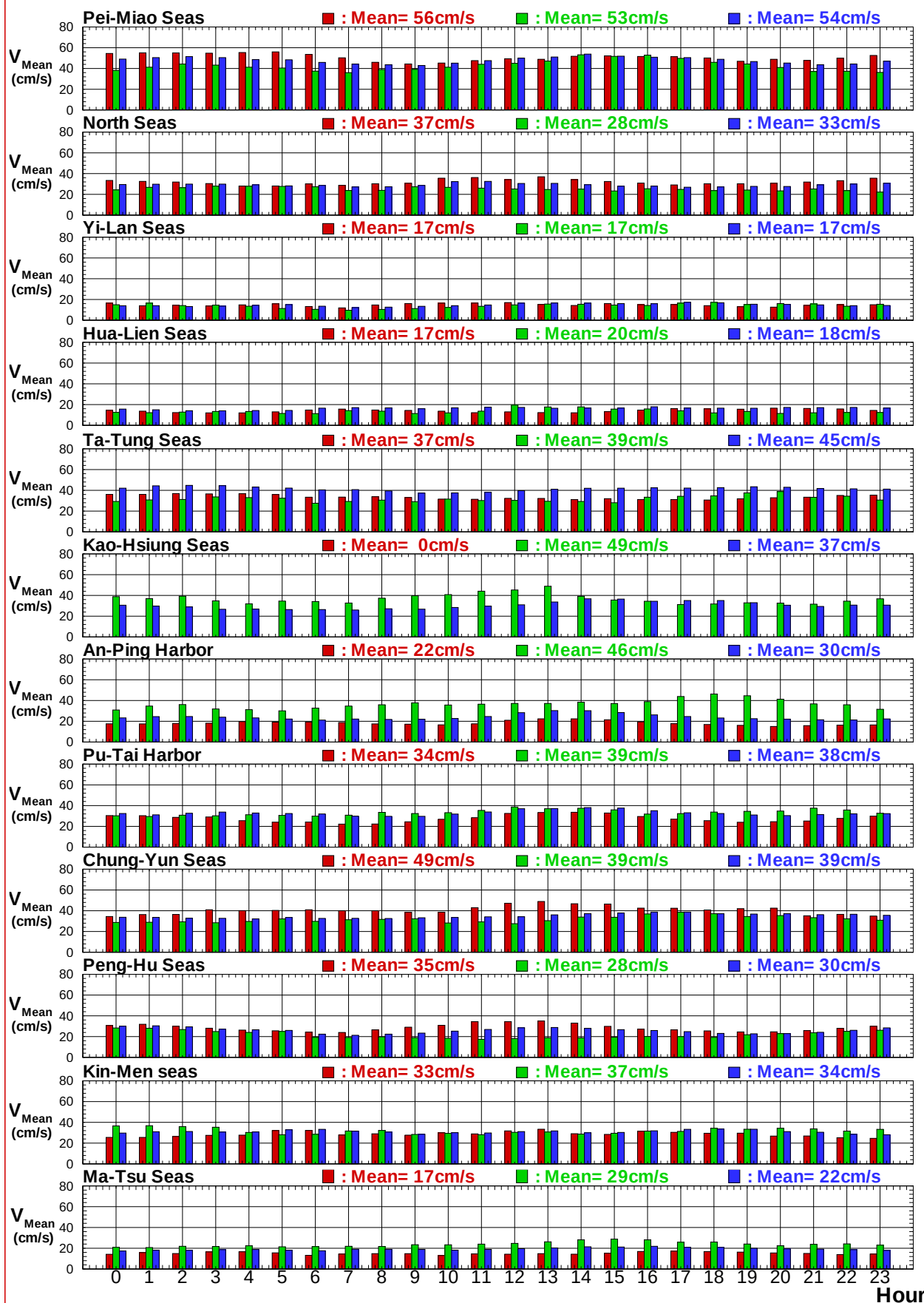
圖7.4a 2018年12港域冬, 夏及整年主要測站逐時平均流速比較圖
