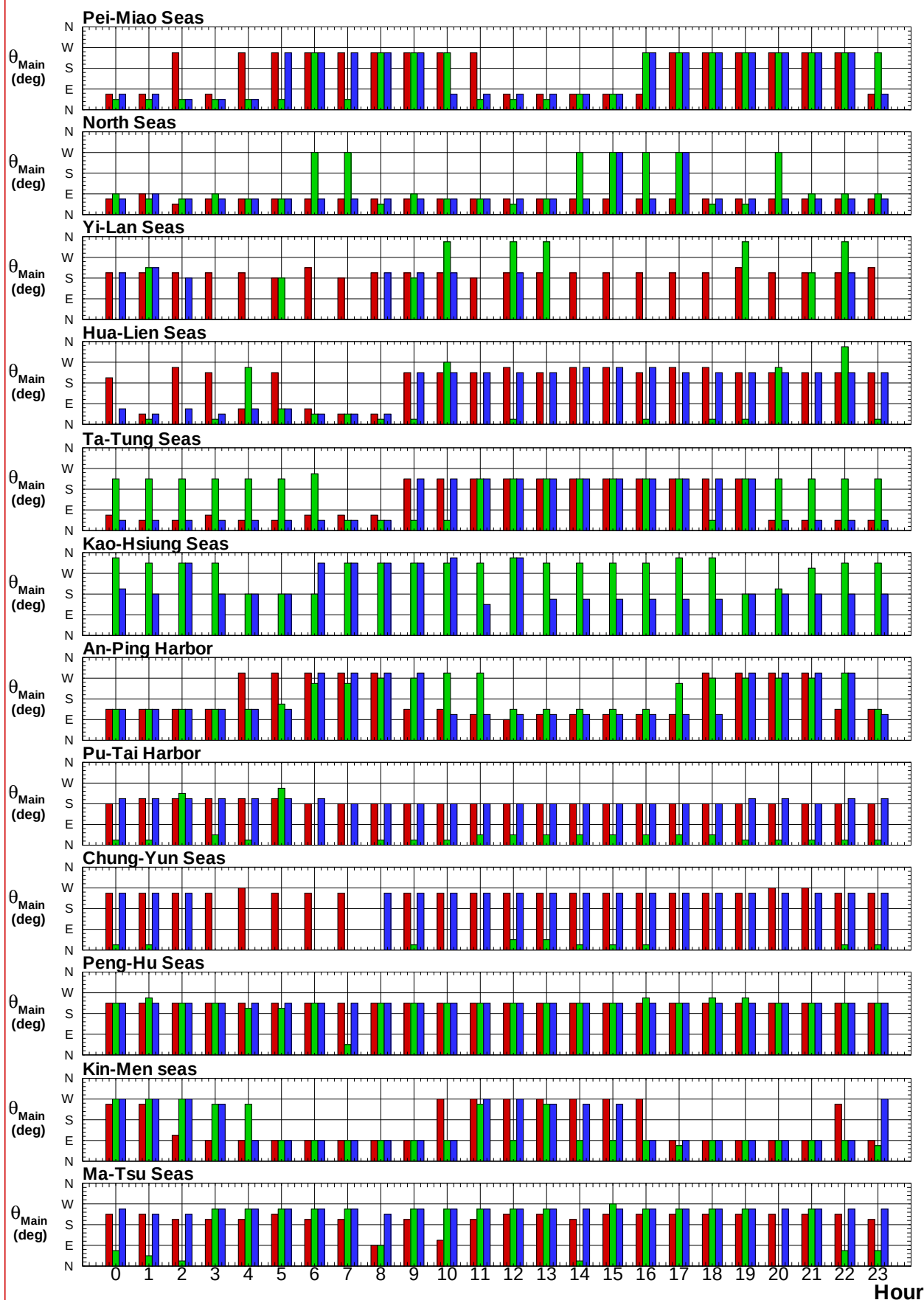
圖7.4e 2018年12港域冬, 夏及整年主要測站逐時主要流向比較圖
