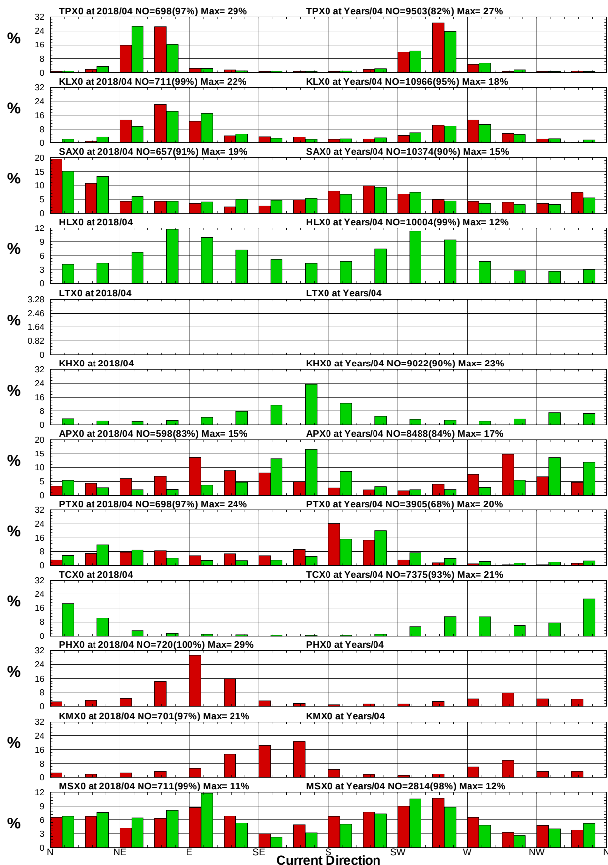
圖8.10 12港域2018年及歷年 4月流向統計方塊圖
