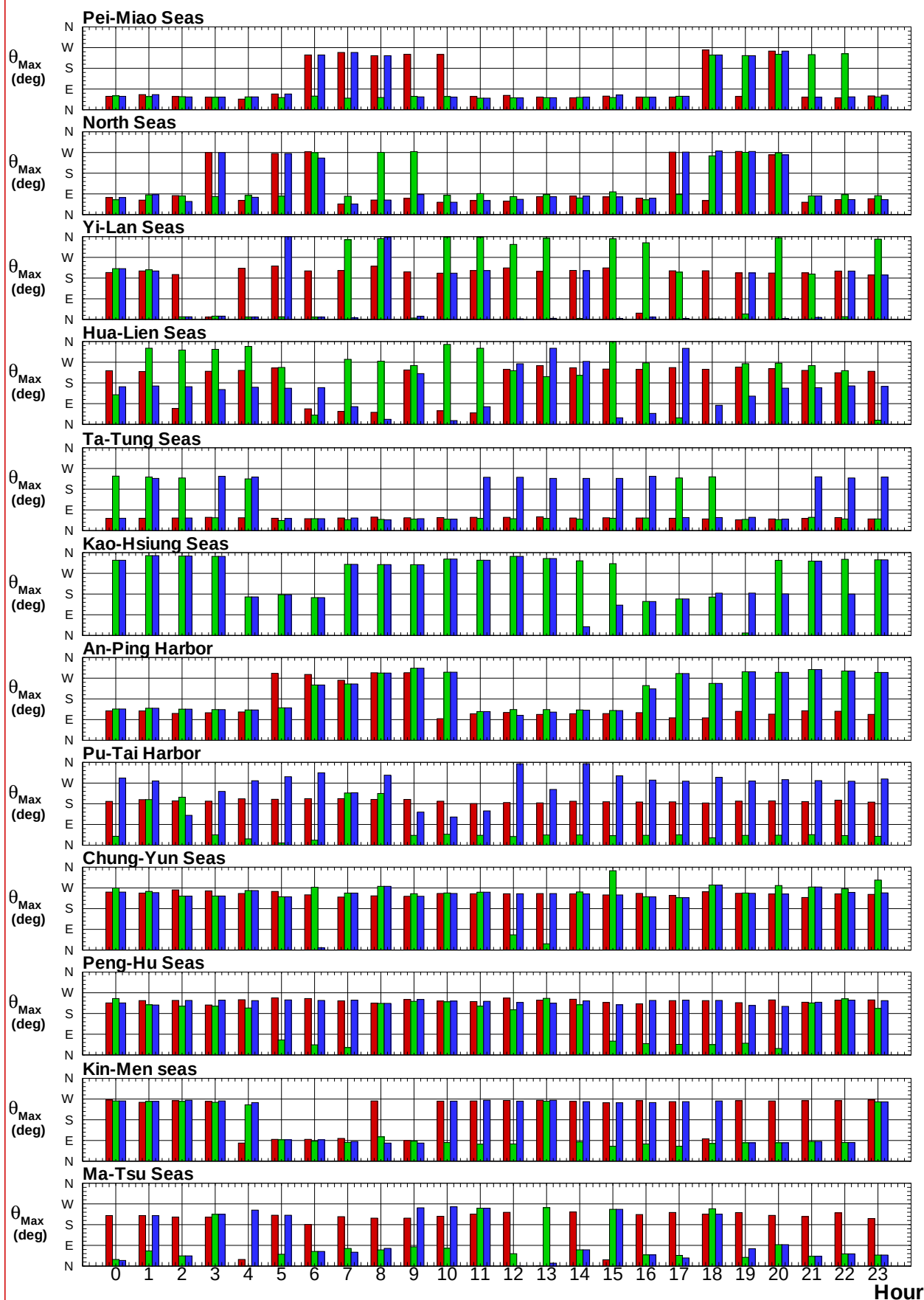
圖7.4d 2018年12港域冬, 夏及整年主要測站逐時最大流速之流向圖
