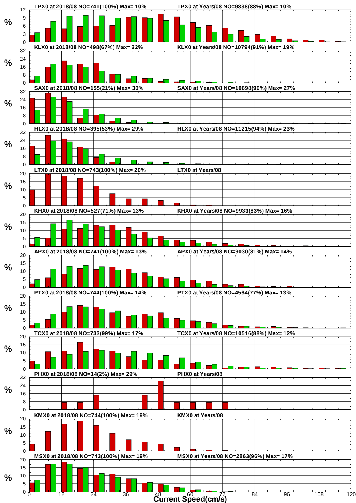
圖8.17 12港域2018年及歷年 8月流速統計方塊圖
