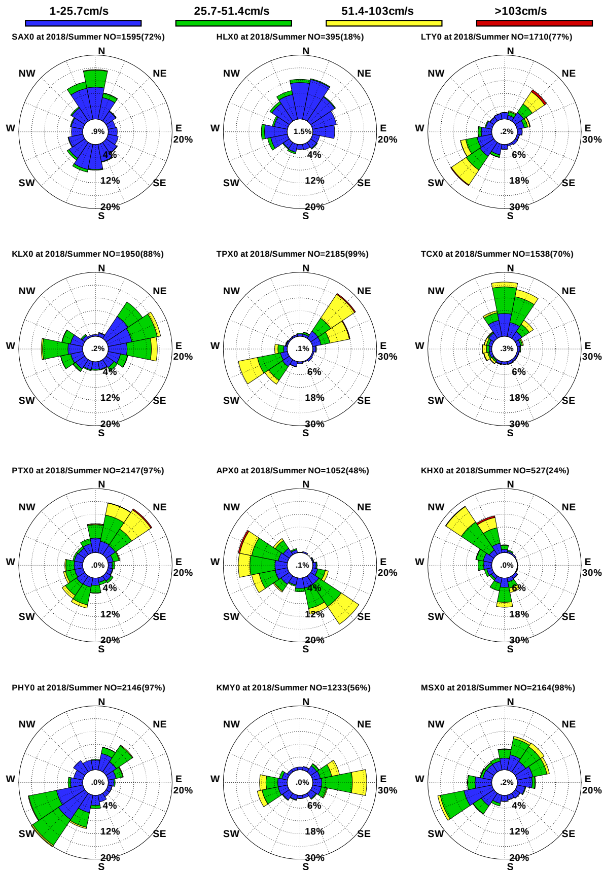
圖9.29 12港域2018年夏季觀測海流玫瑰比較圖
