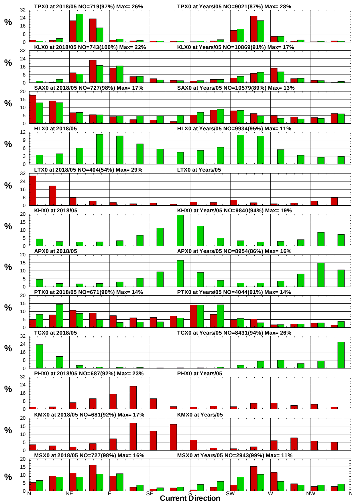
圖8.12 12港域2018年及歷年 5月流向統計方塊圖
