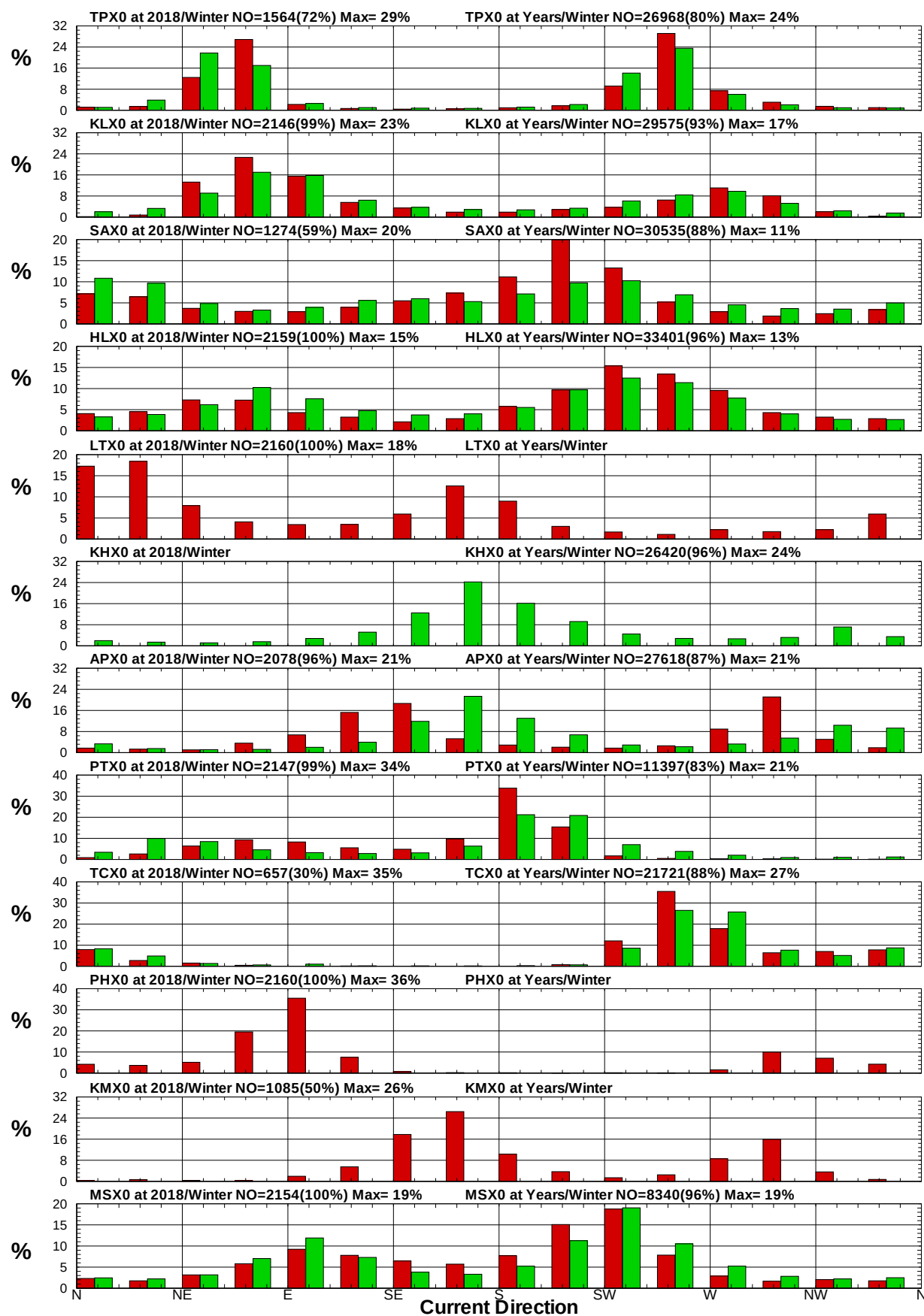
圖8.26 12港域2018年及歷年冬季流向統計方塊圖
