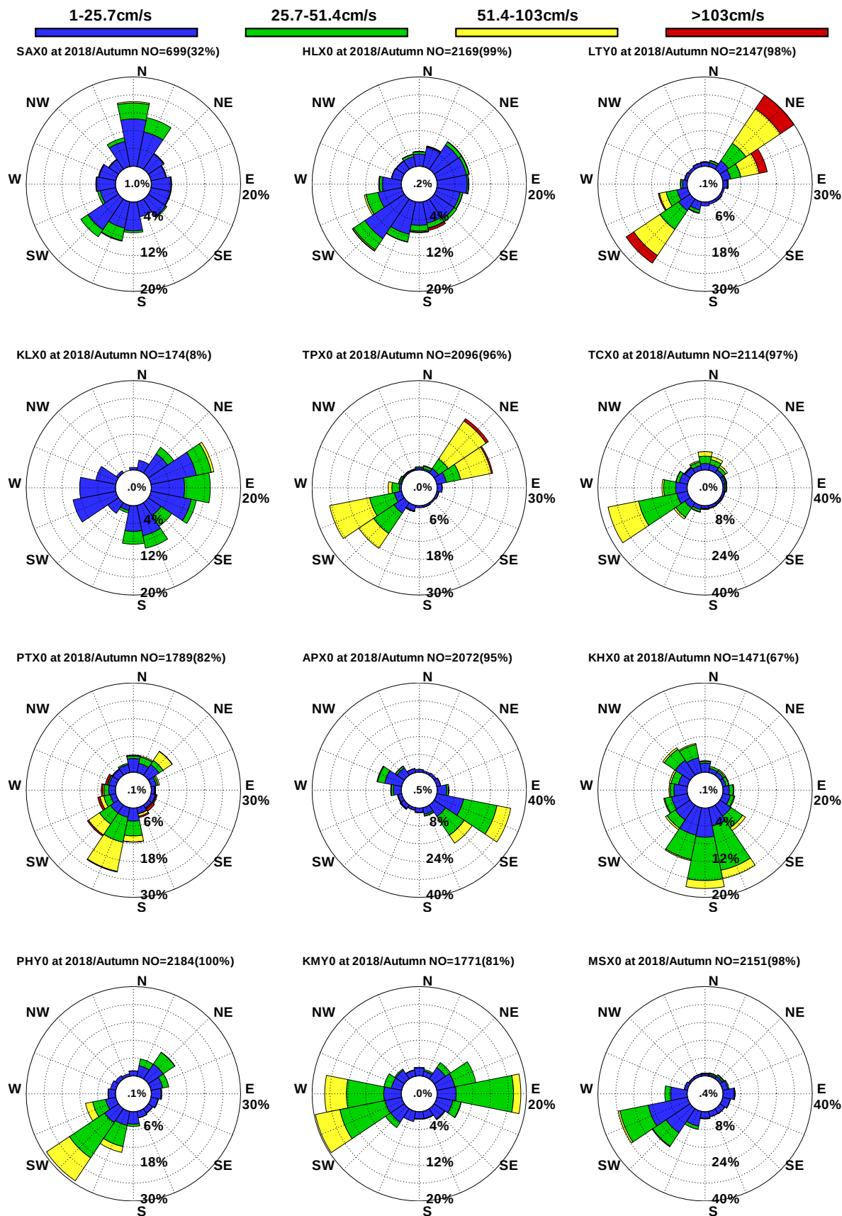
圖9.31 12港域2018年秋季觀測海流玫瑰比較圖
