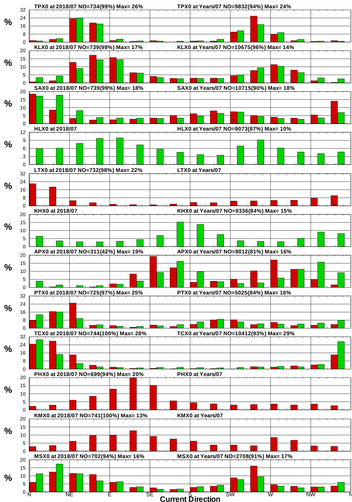
圖8.16 12港域2018年及歷年 7月流向統計方塊圖
