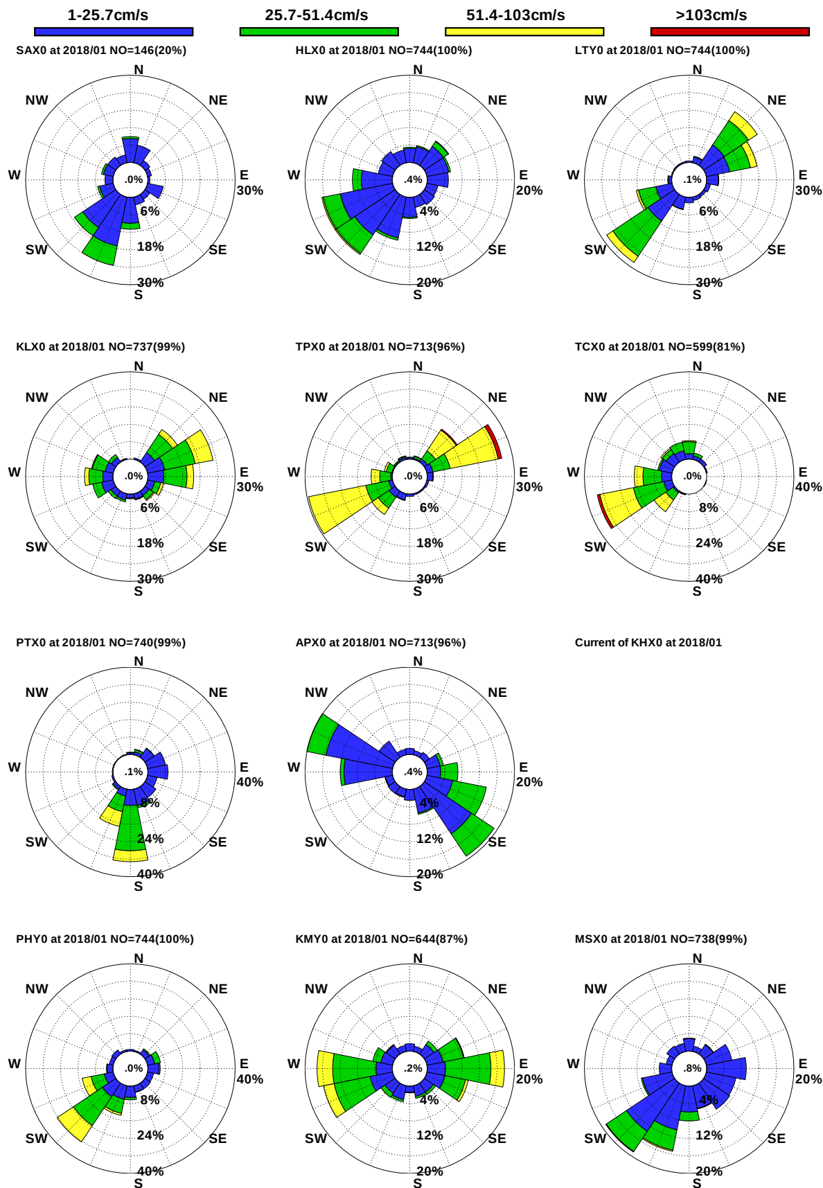
圖9.3 12港域2018年 1月觀測海流玫瑰比較圖
