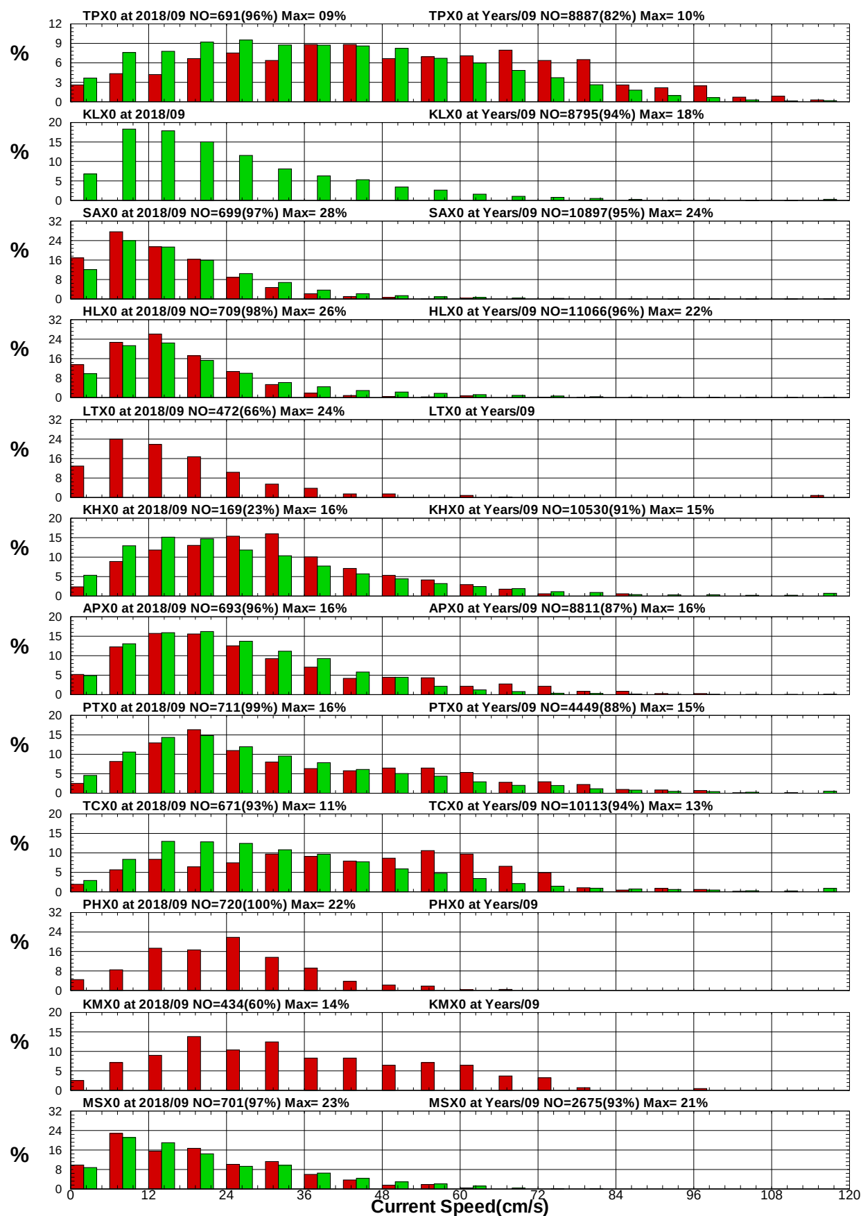
圖8.19 12港域2018年及歷年 9月流速統計方塊圖
