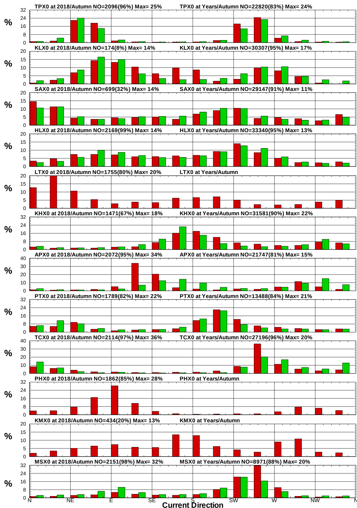
圖8.32 12港域2018年及歷年秋季流向統計方塊圖
