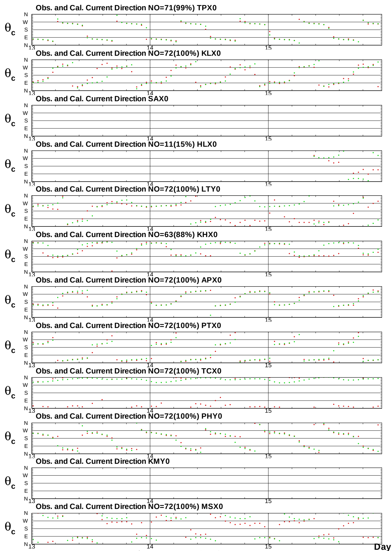
圖10.4 2018年山竹 颱風12海域觀測流向歷線圖 (綠色: 潮流)
