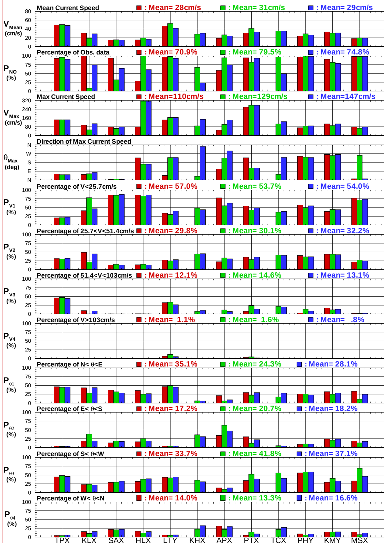
圖7.2c 12個港域2018年主要測站春、秋及整年流速 (向) 比較圖
