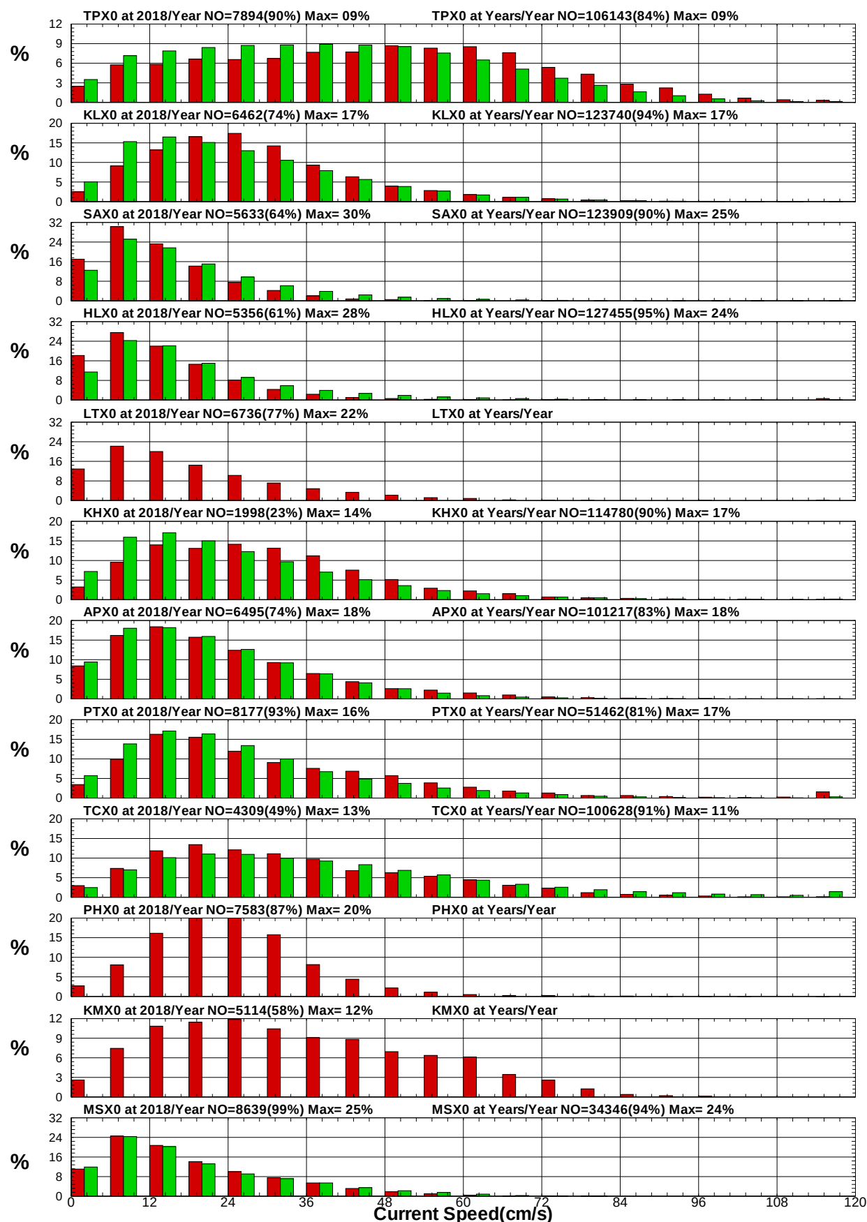
圖8.33 12港域2018年及歷年整年流速統計方塊圖
