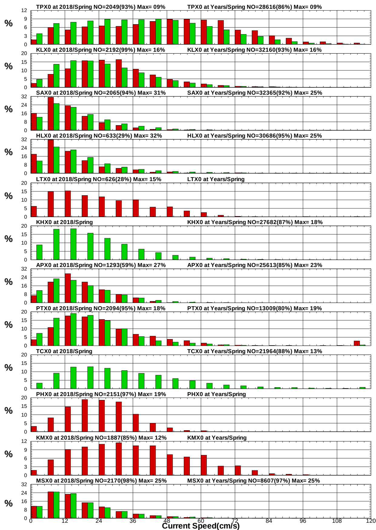
圖8.27 12港域2018年及歷年春季流速統計方塊圖
