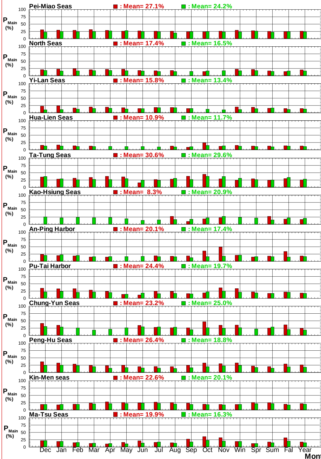
圖7.3f 2018及歷年12港域主要測站每月(季)主要流向百分比圖
