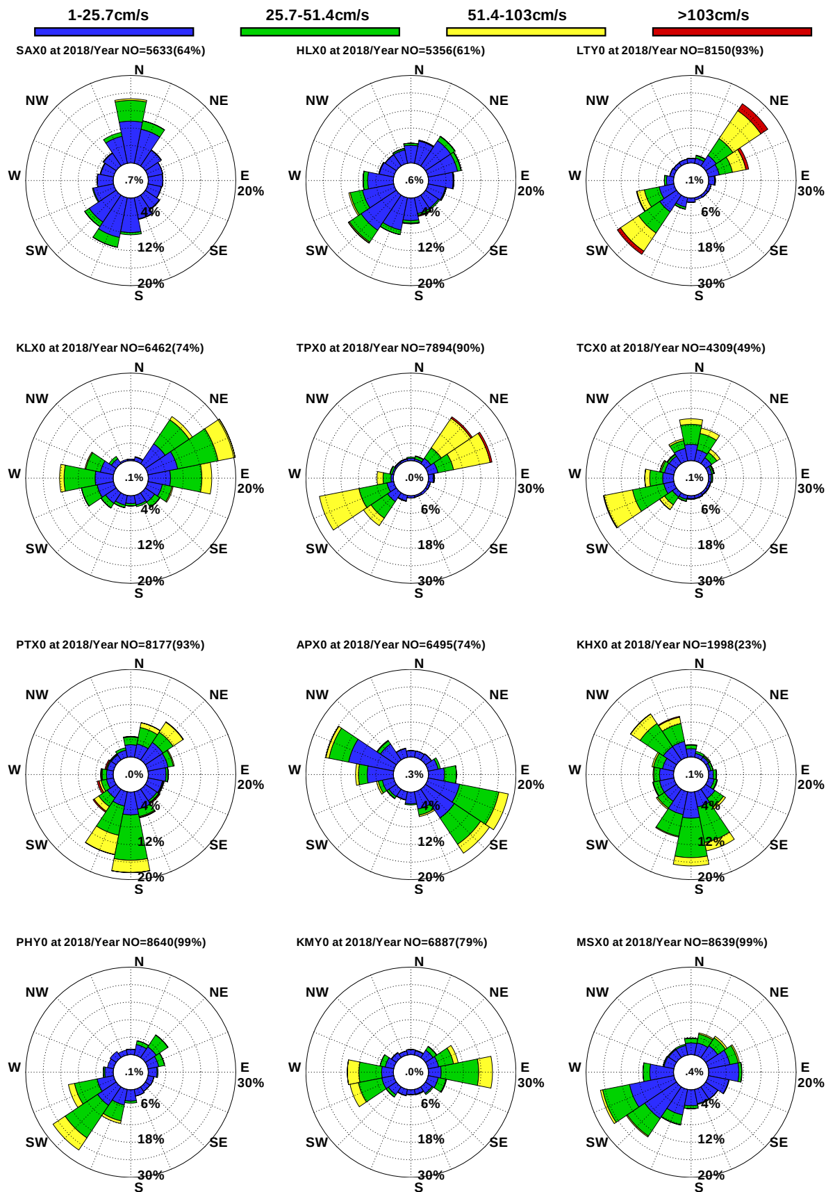
圖9.33 12港域2018年整年觀測海流玫瑰比較圖
