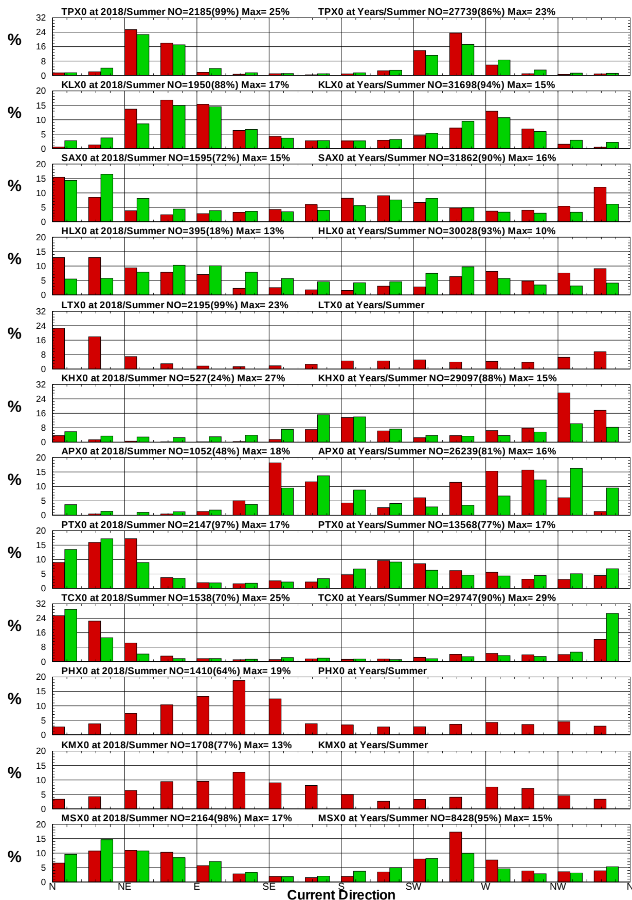
圖8.30 12港域2018年及歷年夏季流向統計方塊圖
