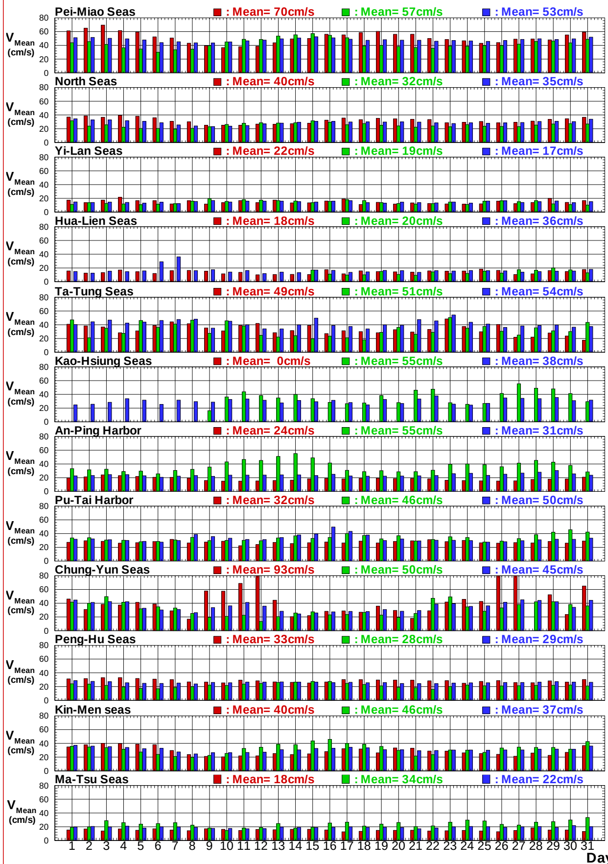
圖7.6a 2018年12港域冬, 夏及整年主要測站每日平均流速比較圖
