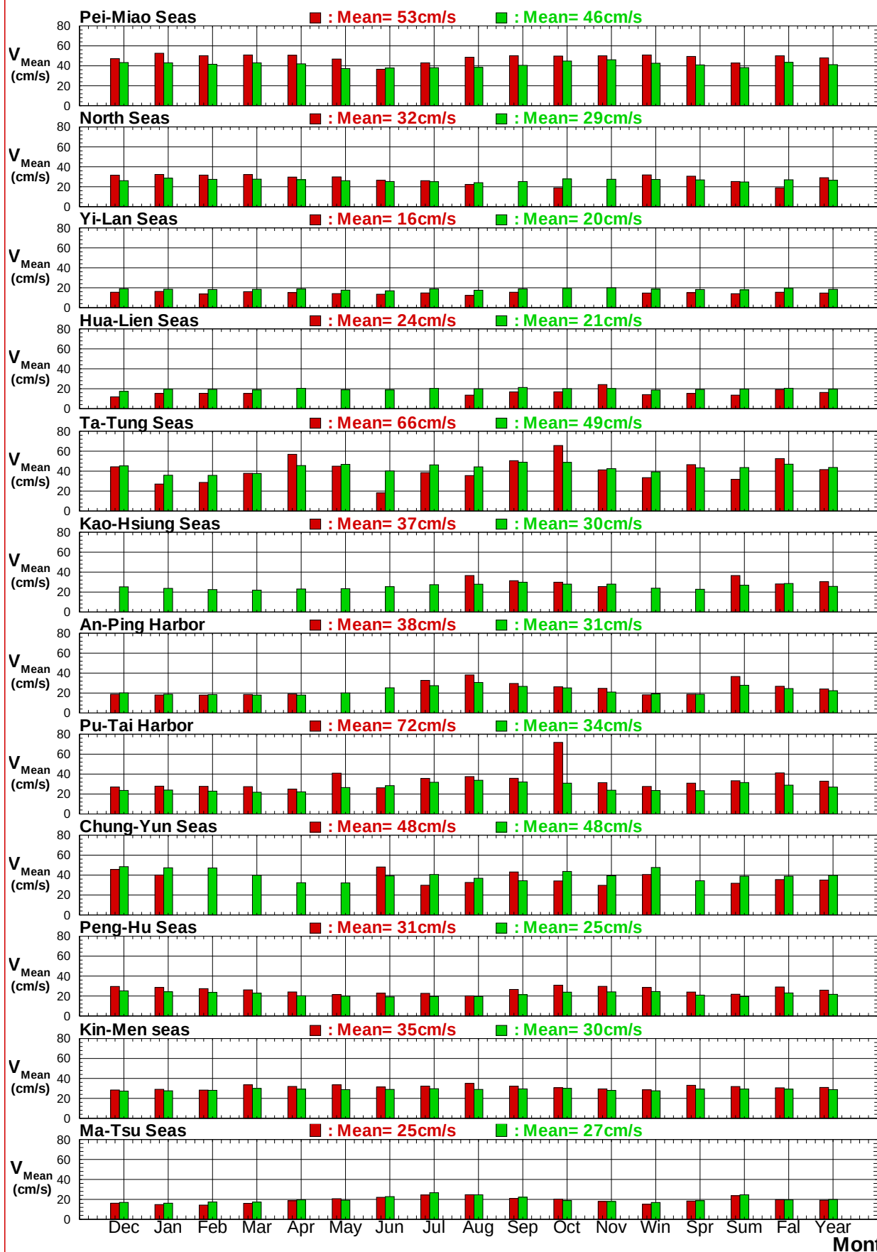
圖7.3a 2018及歷年12港域主要測站每月(季) 平均流速比較圖
