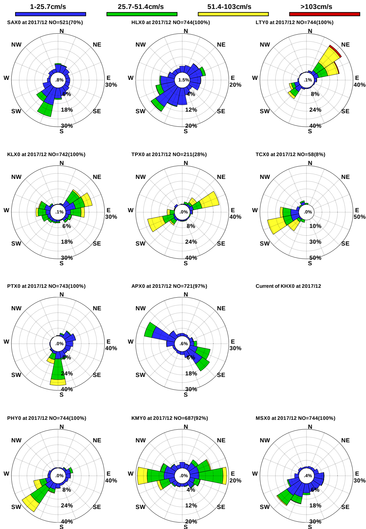
圖9.1 12港域2017年12月觀測海流玫瑰比較圖
