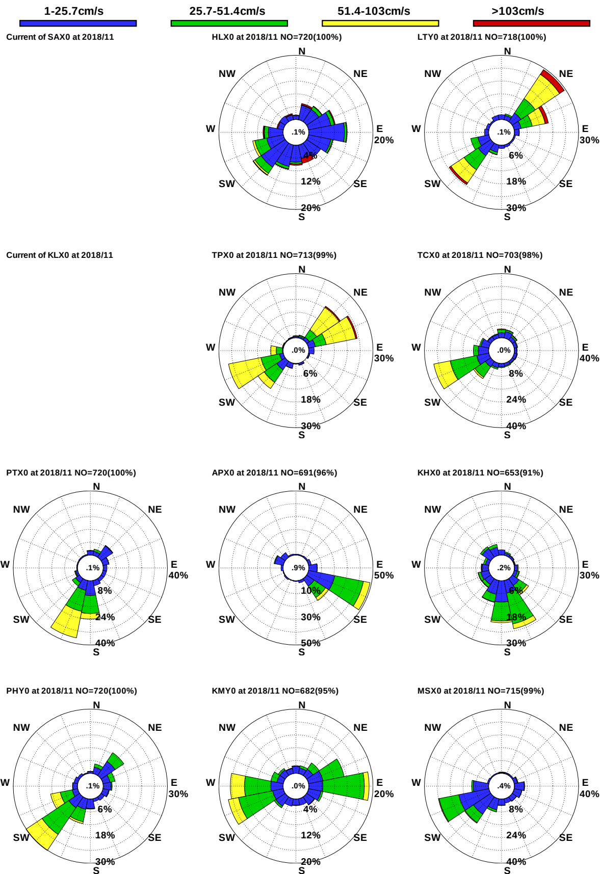
圖9.23 12港域2018年11月觀測海流玫瑰比較圖
