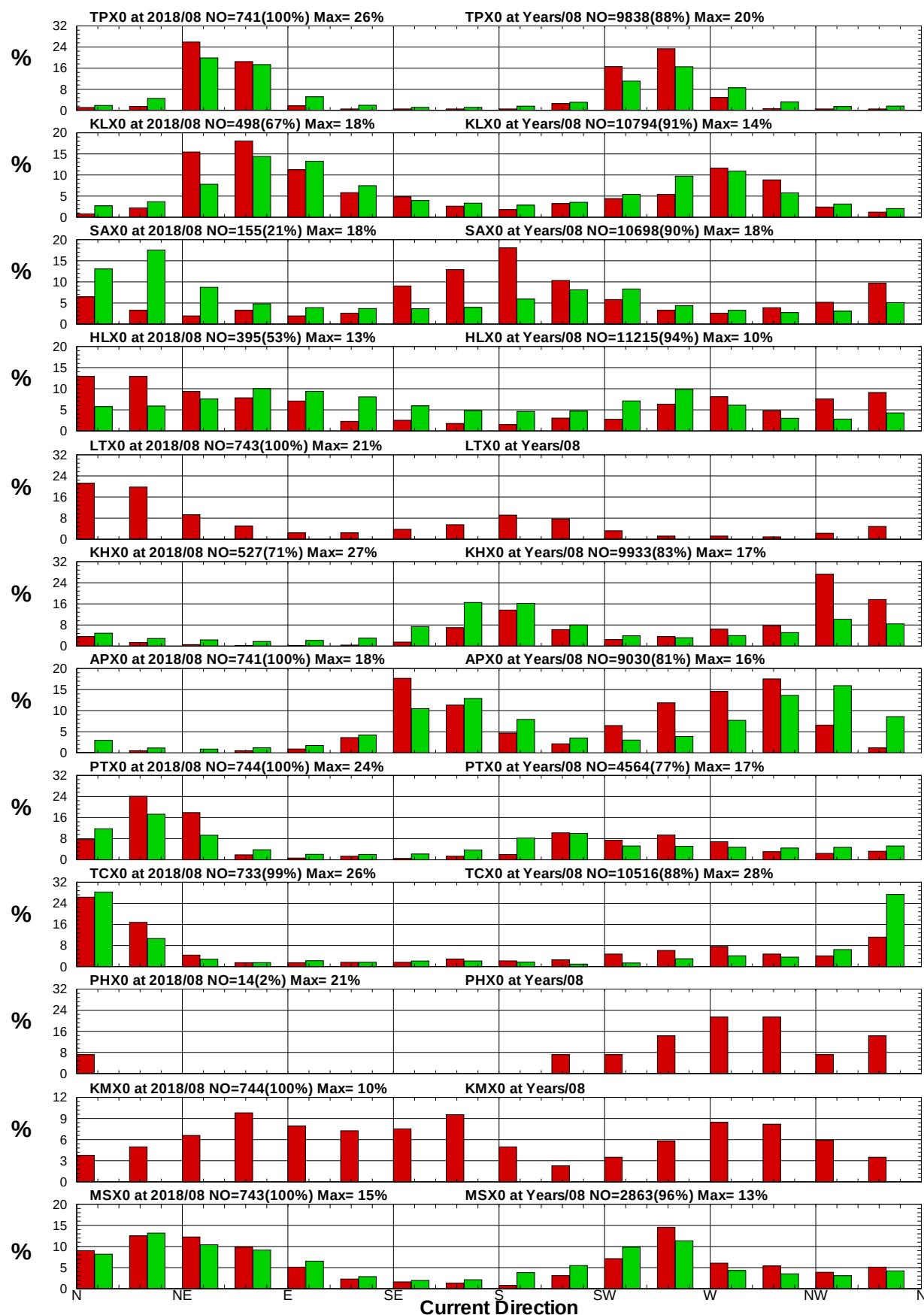
圖8.18 12港域2018年及歷年 8月流向統計方塊圖
