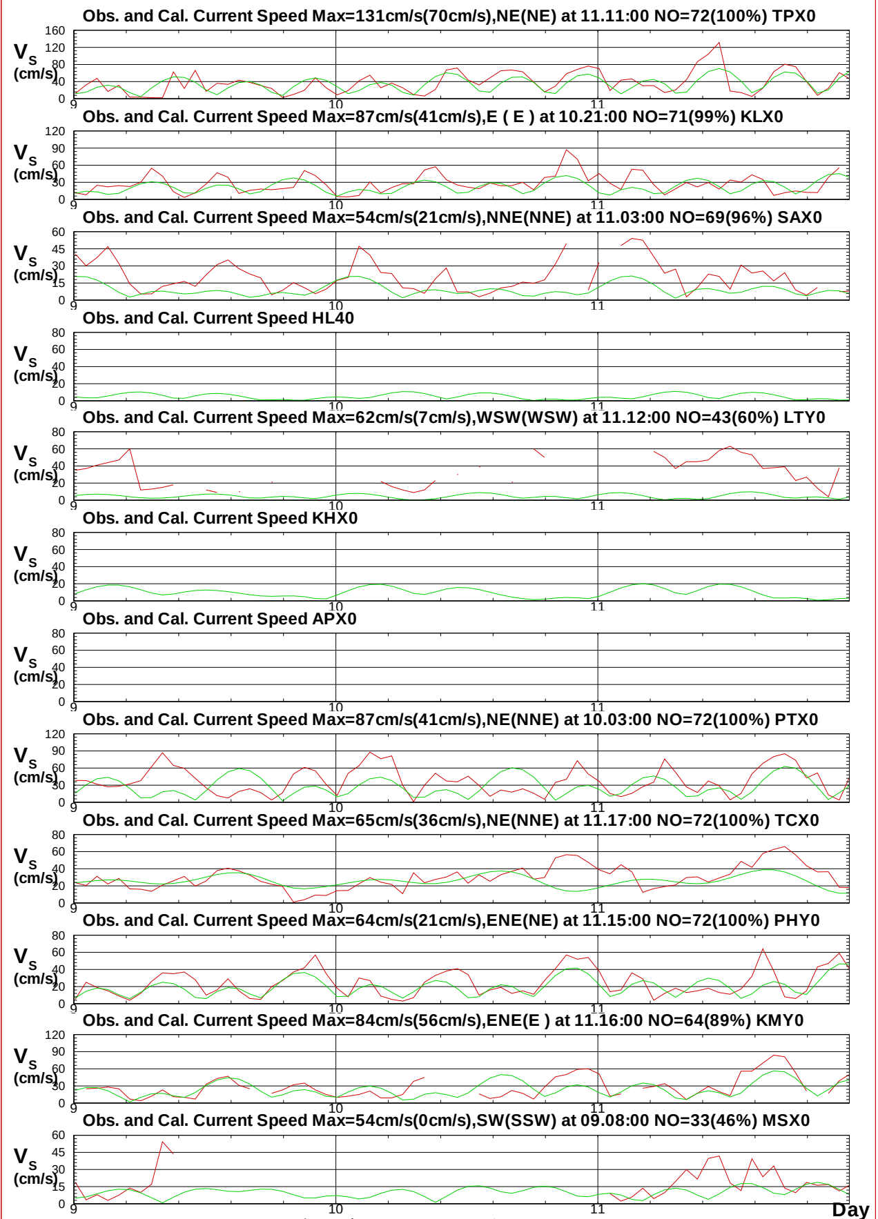
圖10.1 2018年瑪莉亞颱風12海域觀測流速歷線圖 (綠色: 潮流)
