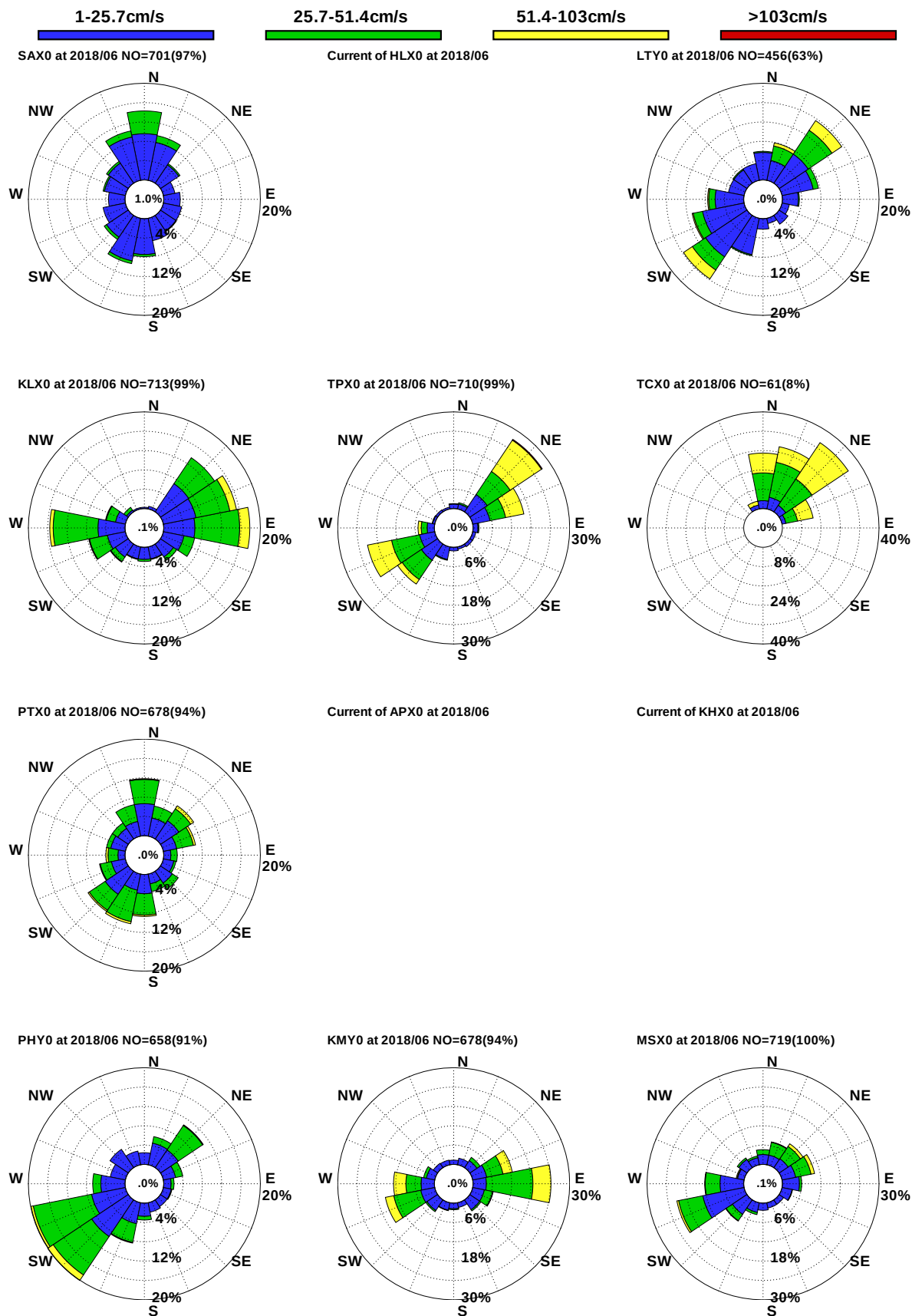
圖9.13 12港域2018年 6月觀測海流玫瑰比較圖
