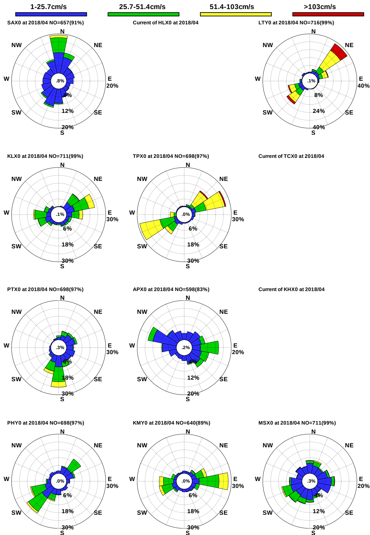
圖9.9 12港域2018年4月觀測海流玫瑰比較圖
