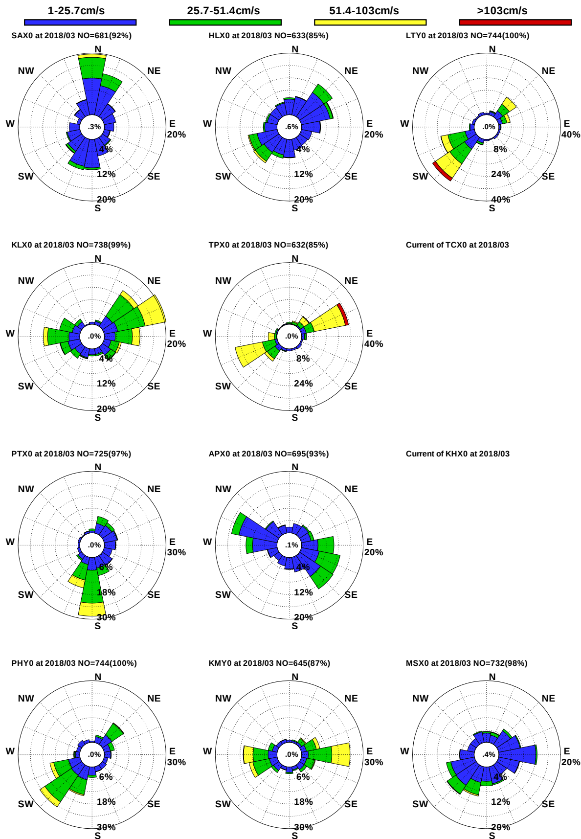
圖9.7 12港域2018年3月觀測海流玫瑰比較圖
