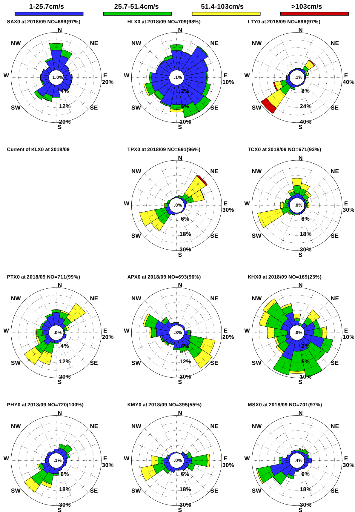
圖9.19 12港域2018年 9月觀測海流玫瑰比較圖
