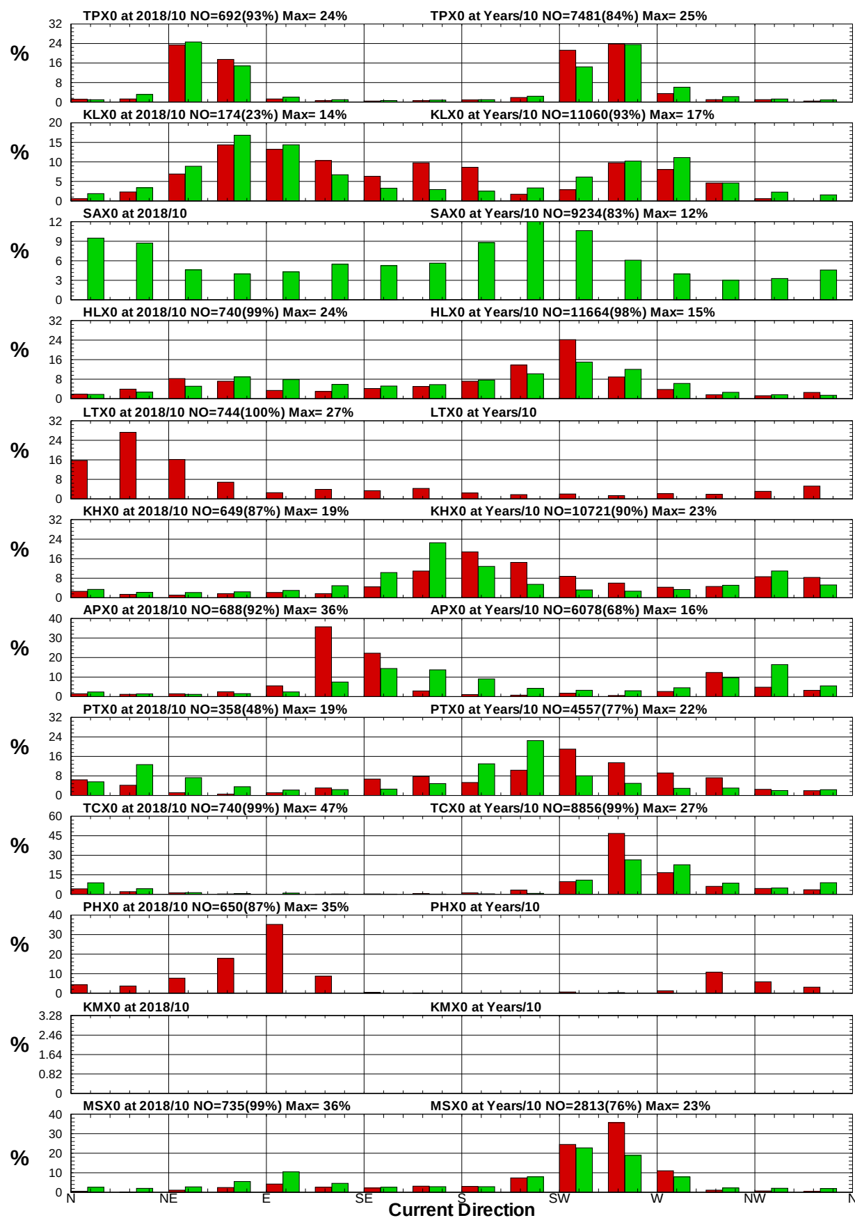
圖8.22 12港域2018年及歷年10月流向統計方塊圖
