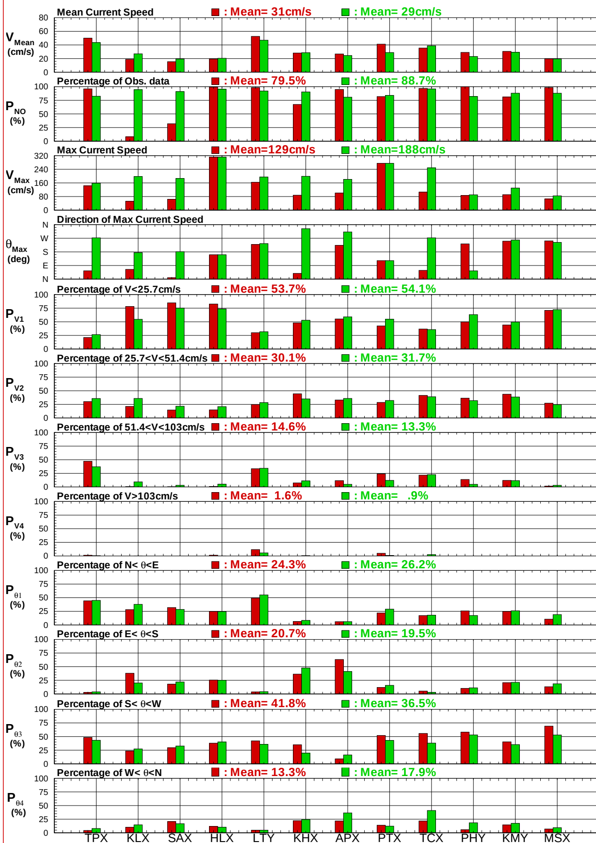
圖7.1d 12個港域2018及歷年主要測站秋季流速(向)比較圖
