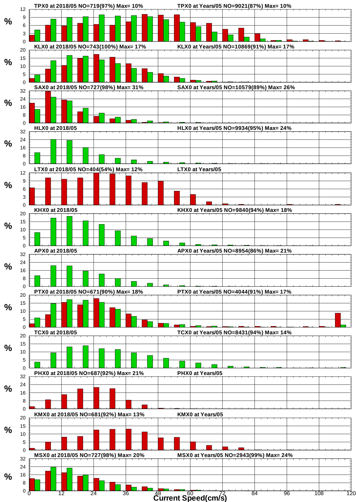
圖8.11 12港域2018年及歷年5月流速統計方塊圖
