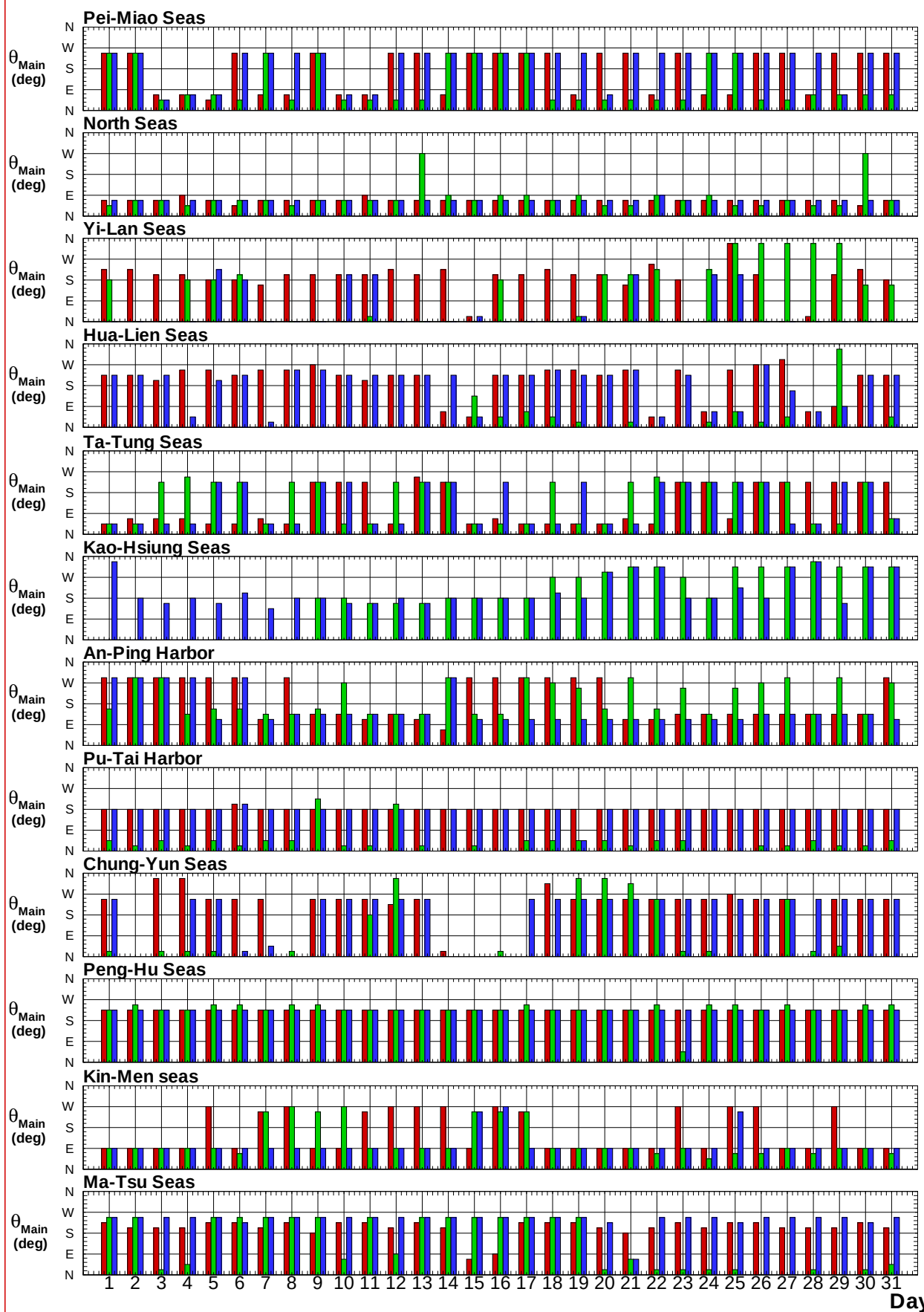
圖7.6e 2018年12港域冬, 夏及整年主要測站每日主要流向比較圖
