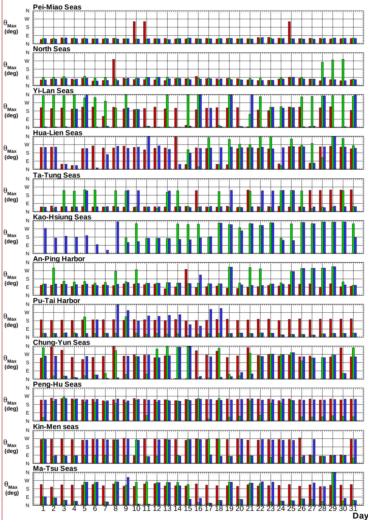
圖 7.6d 2018 年 12 港域冬, 夏及整年主要測站每日最大流速之流向圖
