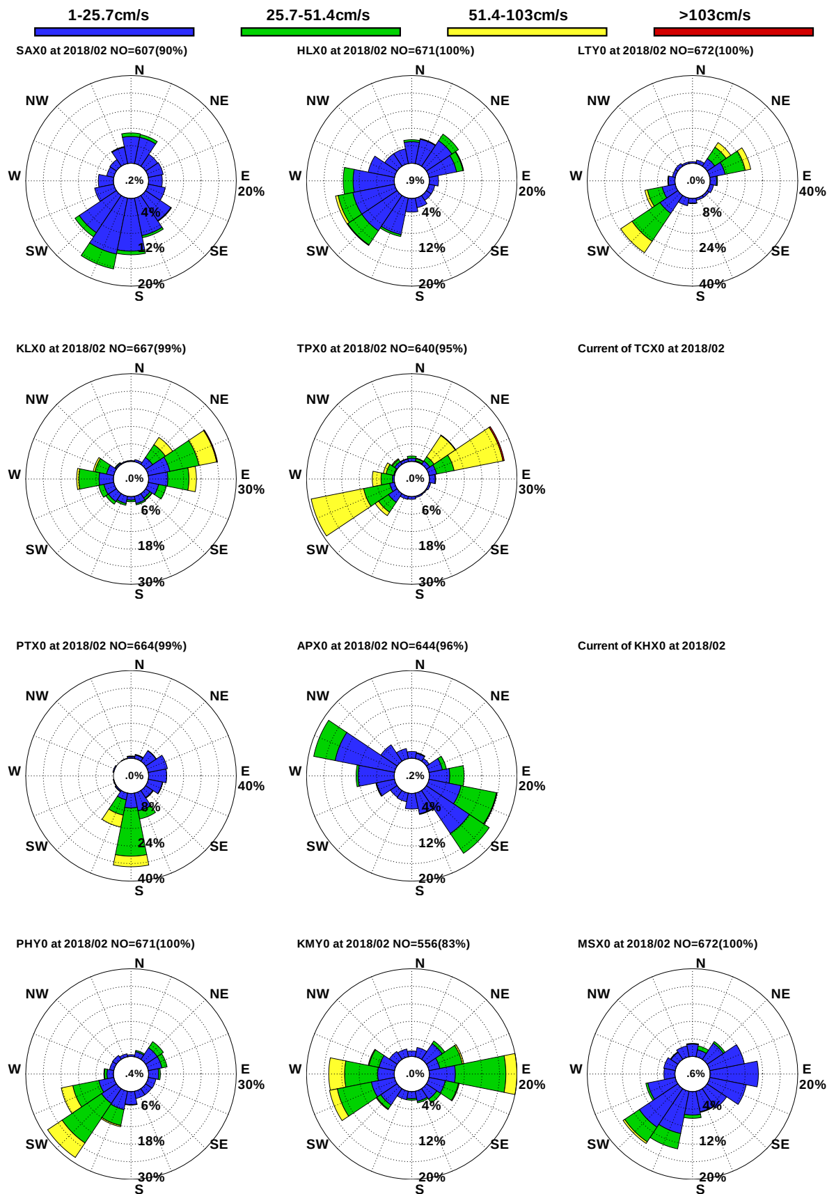
圖9.5 12港域2018年2月觀測海流玫瑰比較圖
