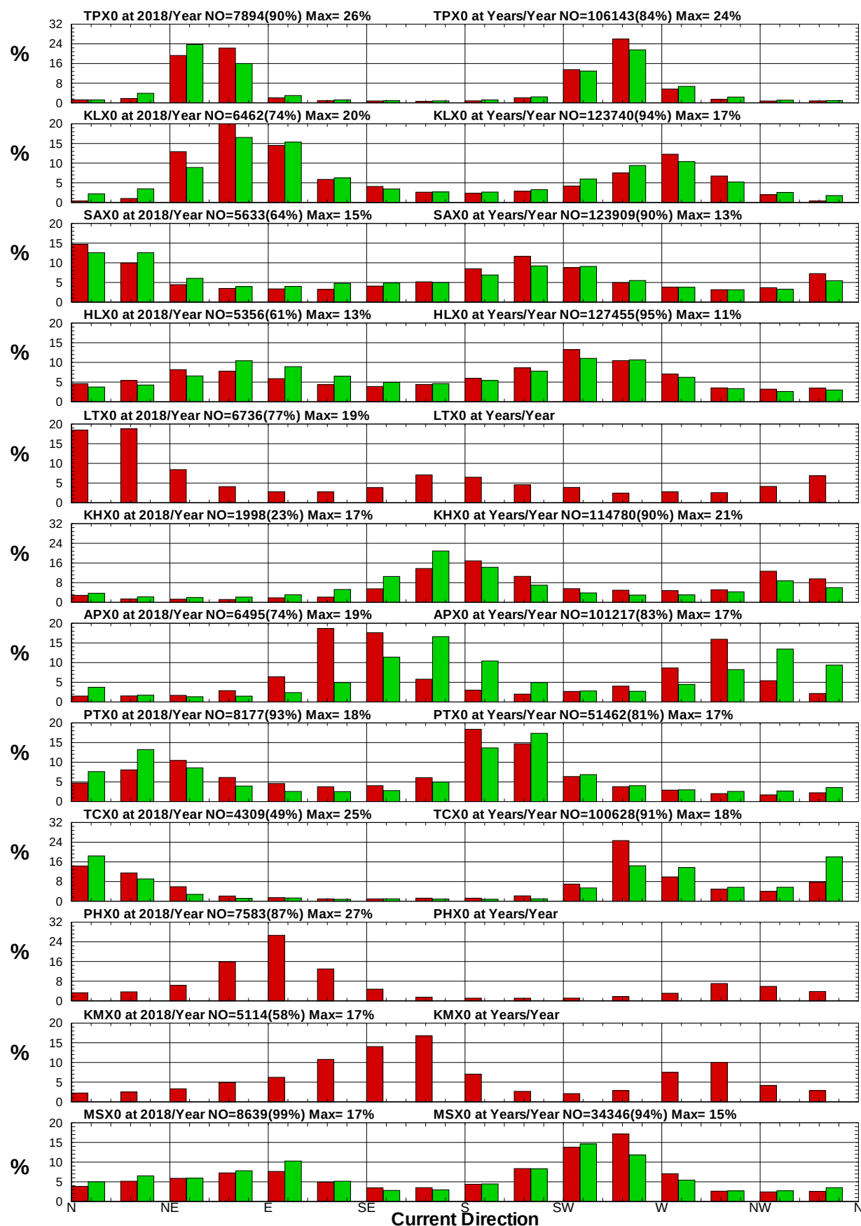
圖8.34 12港域2018年及歷年整年流向統計方塊圖
