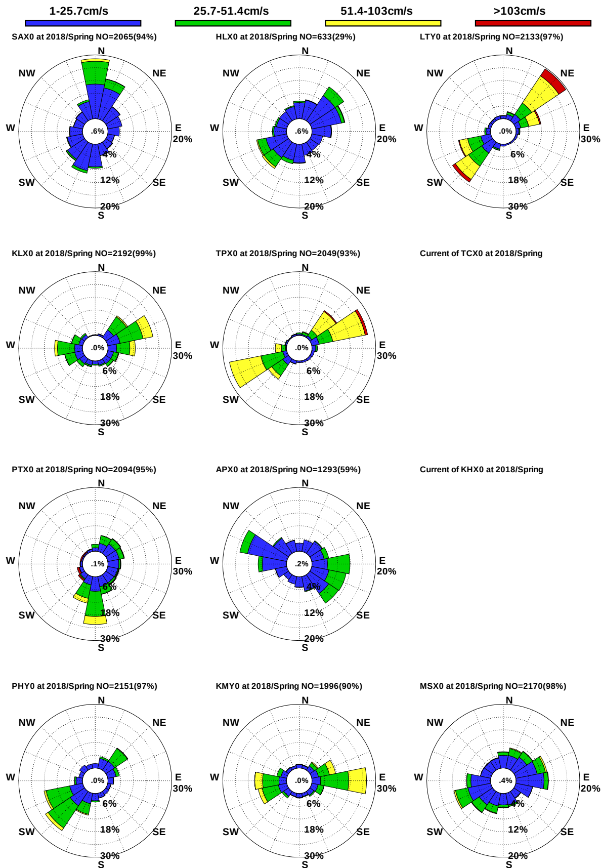
圖9.27 12港域2018年春季觀測海流玫瑰比較圖
