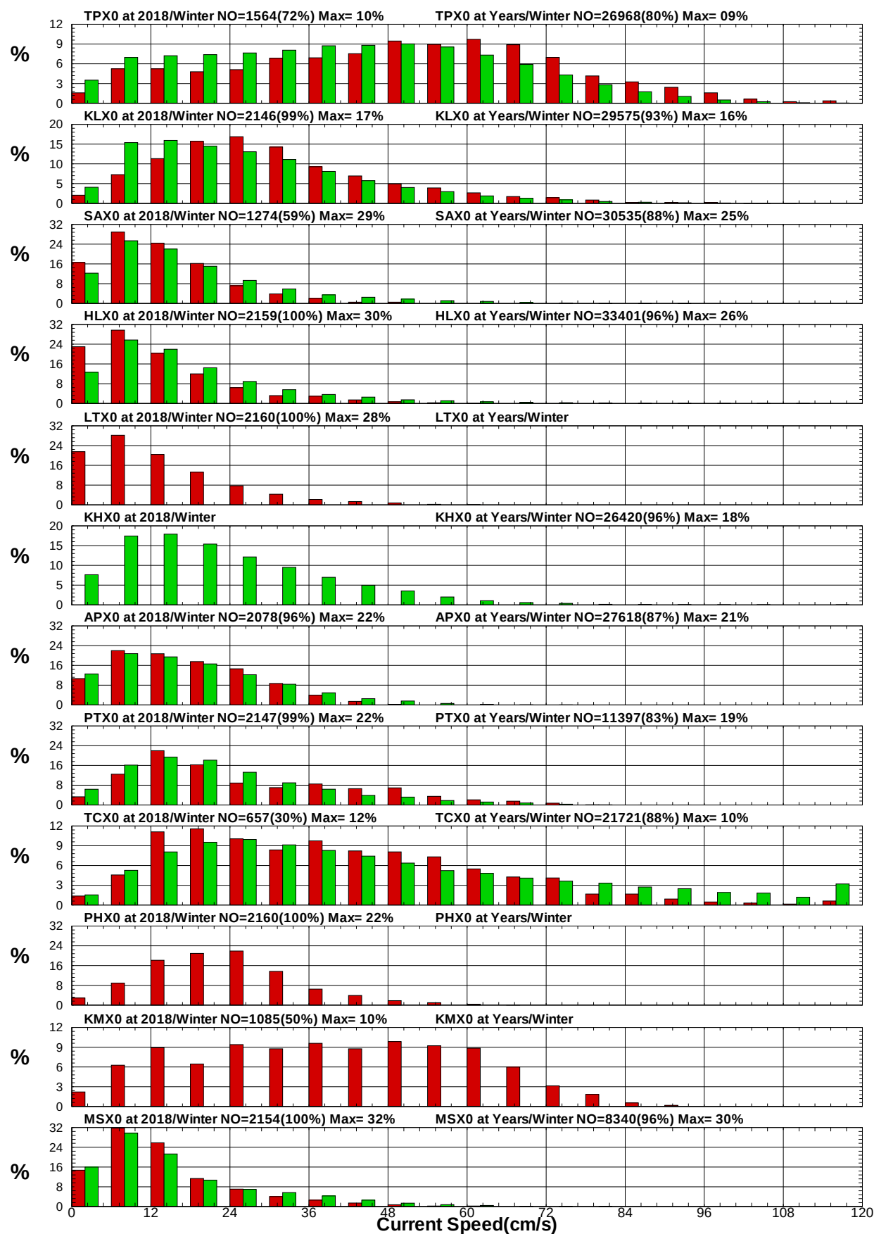
圖8.25 12港域2018年及歷年冬季流速統計方塊圖
