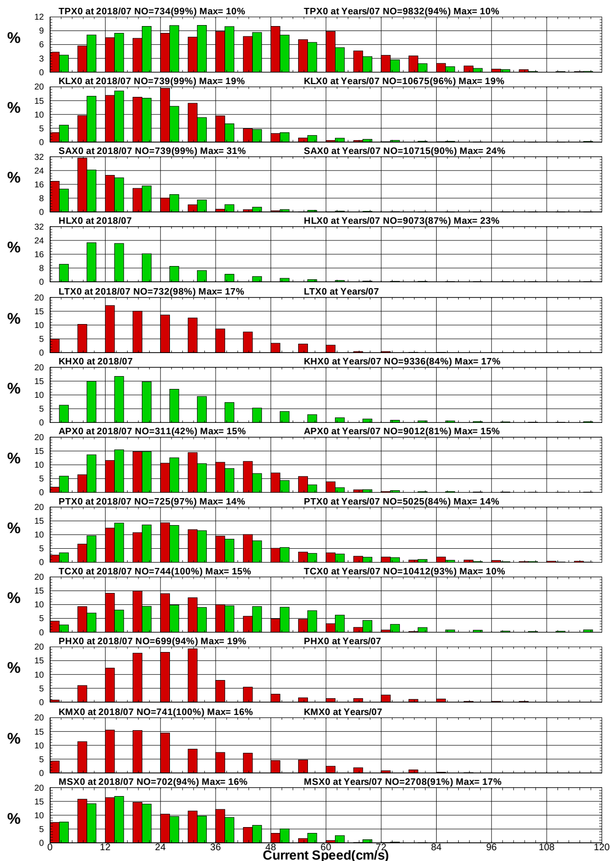
圖8.15 12港域2018年及歷年 7月流速統計方塊圖
