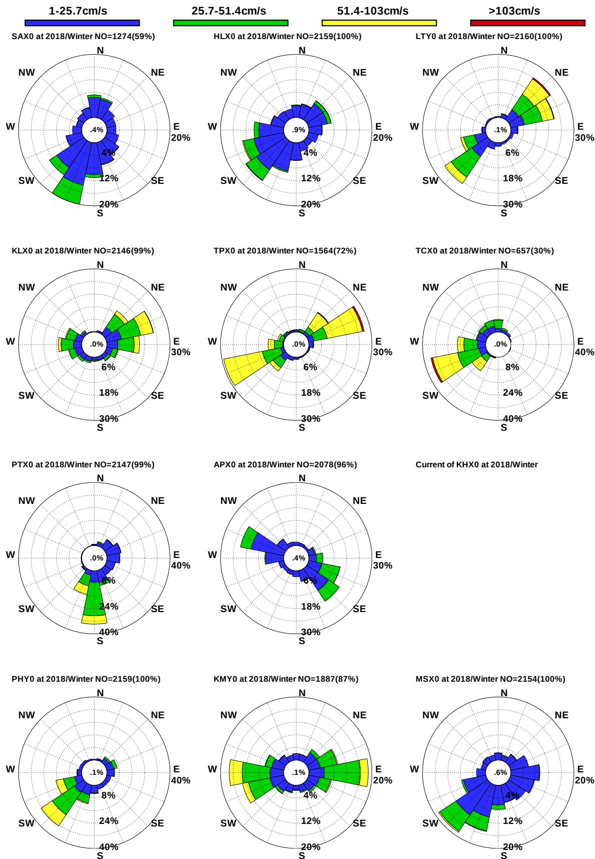
圖9.25 12港域2018年冬季觀測海流玫瑰比較圖
