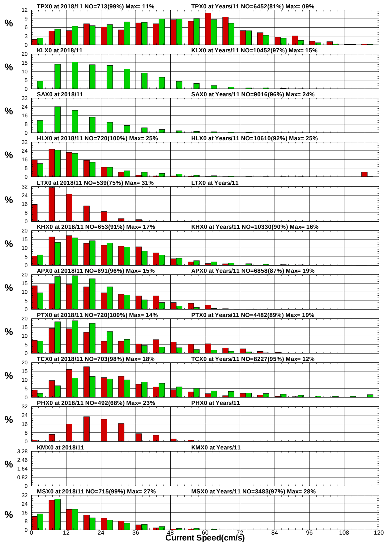
圖8.23 12港域2018年及歷年11月流速統計方塊圖
