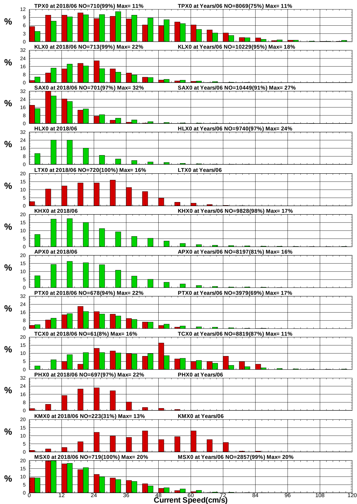
圖8.13 12港域2018年及歷年 6月流速統計方塊圖
