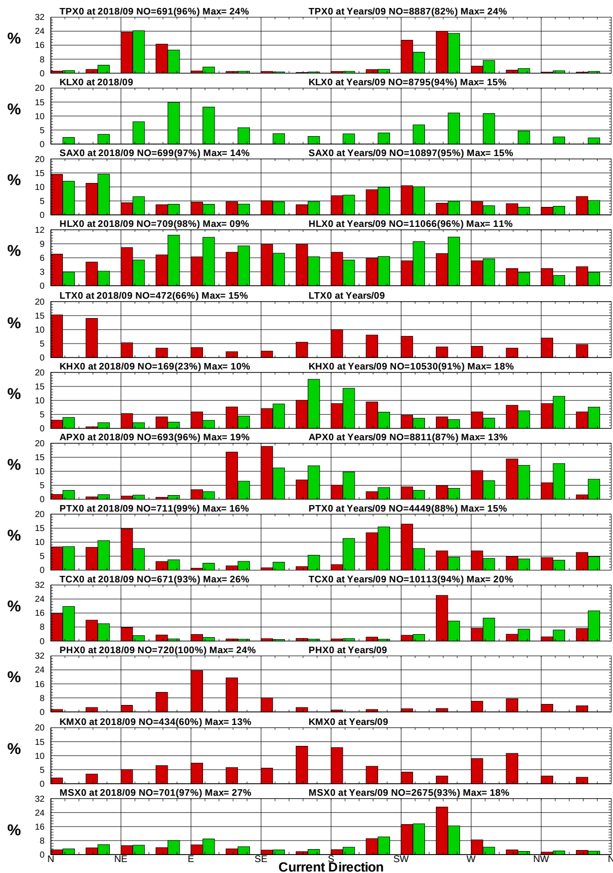
圖8.20 12港域2018年及歷年 9月流向統計方塊圖
