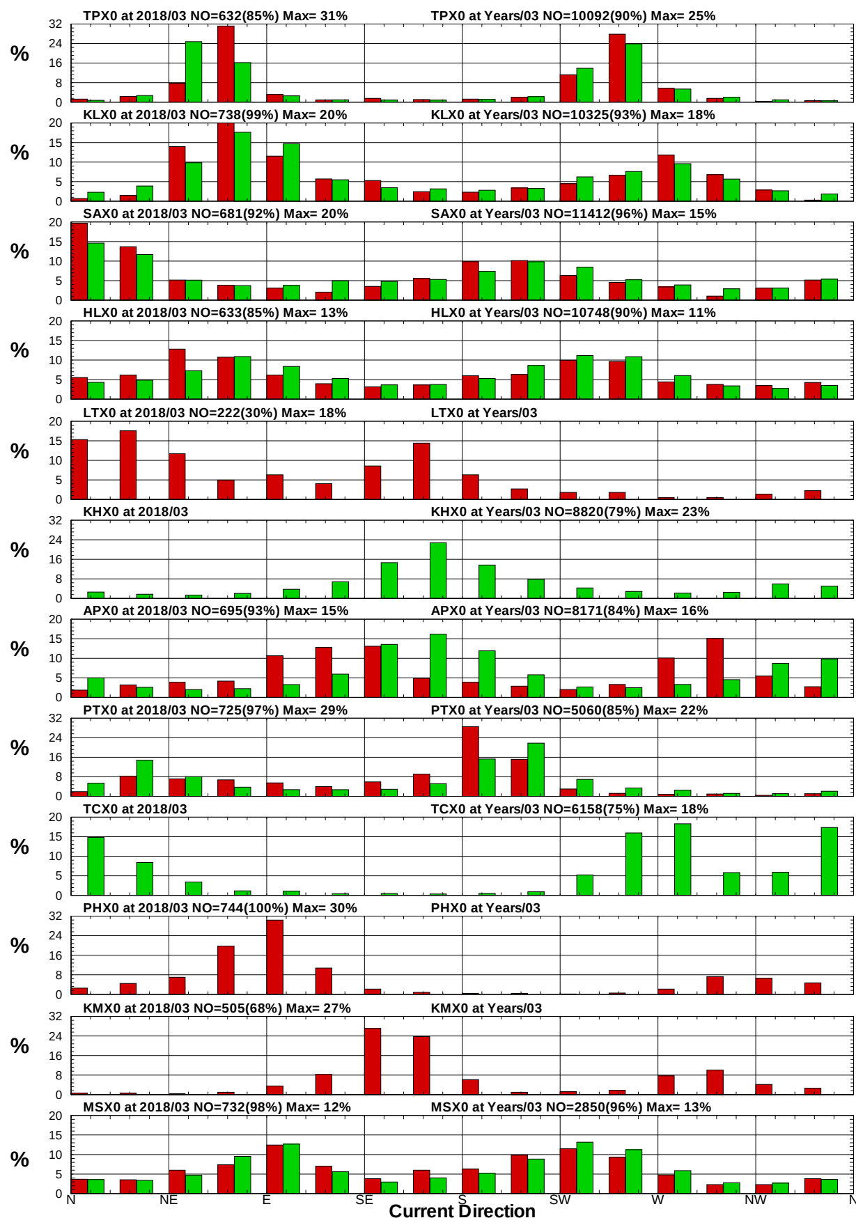
圖8.8 12港域2018年及歷年 3月流向統計方塊圖
