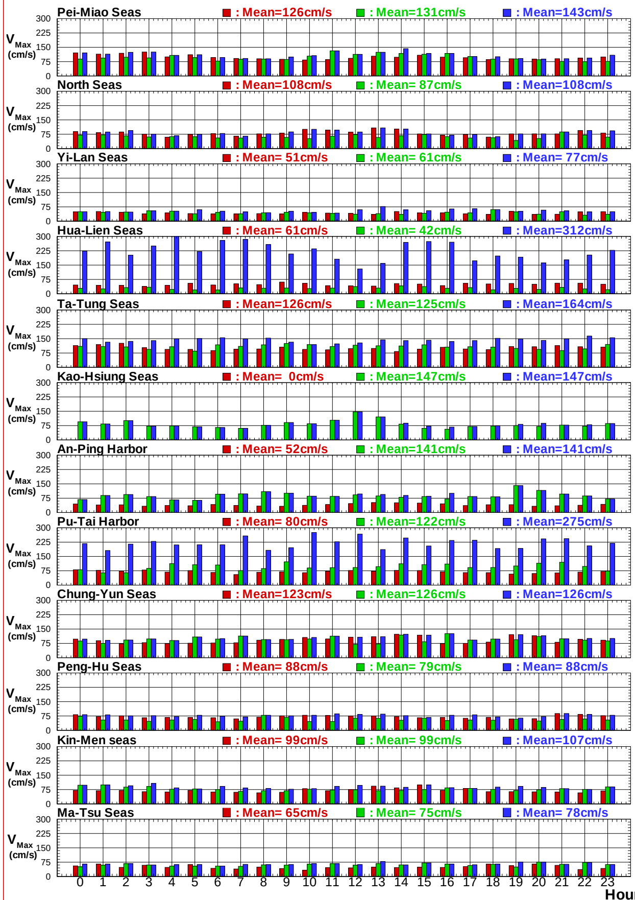
圖7.4c 2018年12港域冬, 夏及整年主要測站逐時最大流速比較圖
