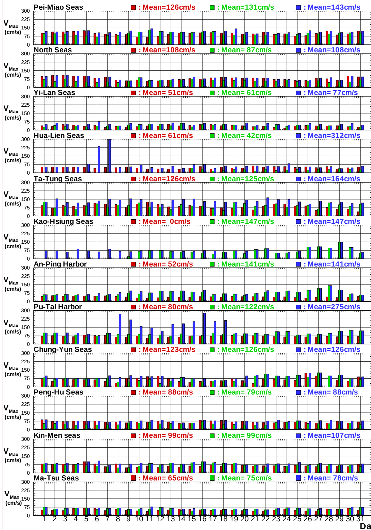
圖7.6c 2018年12港域冬、夏及整年主要測站每日最大流速比較圖
