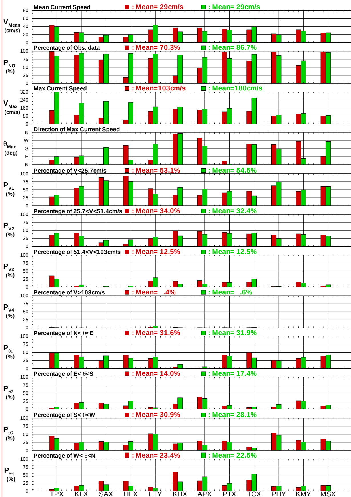
圖7.1c 12個港域2018及歷年主要測站夏季流速(向)比較圖
