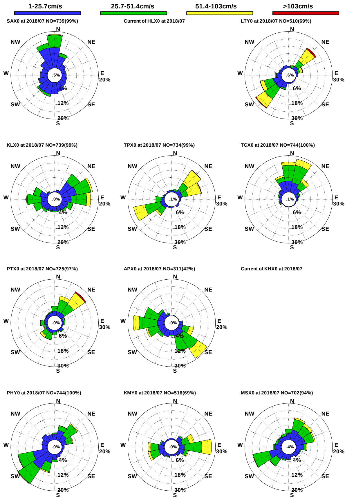
圖9.15 12港域2018年 7月觀測海流玫瑰比較圖
