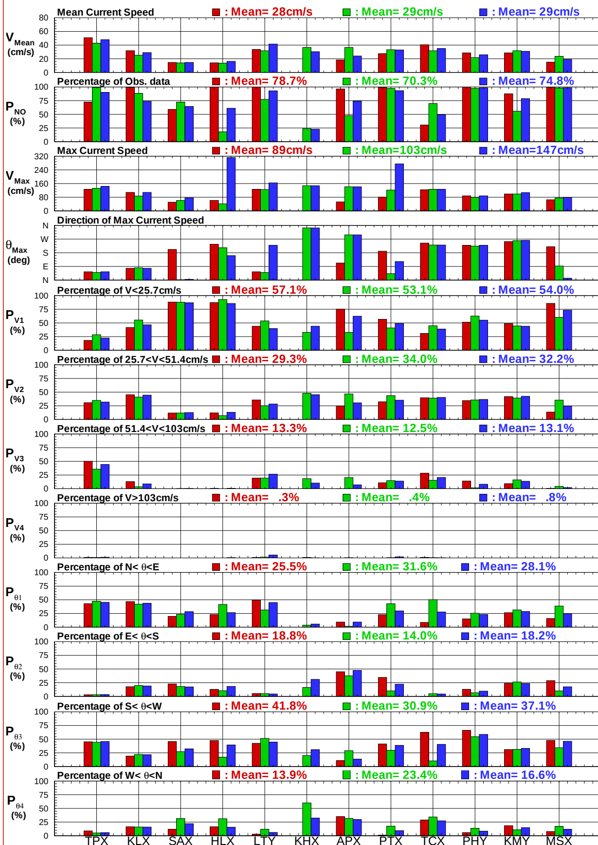
圖7.2a 12個港域2018年主要測站冬, 夏及整年流速 (向) 比較圖
