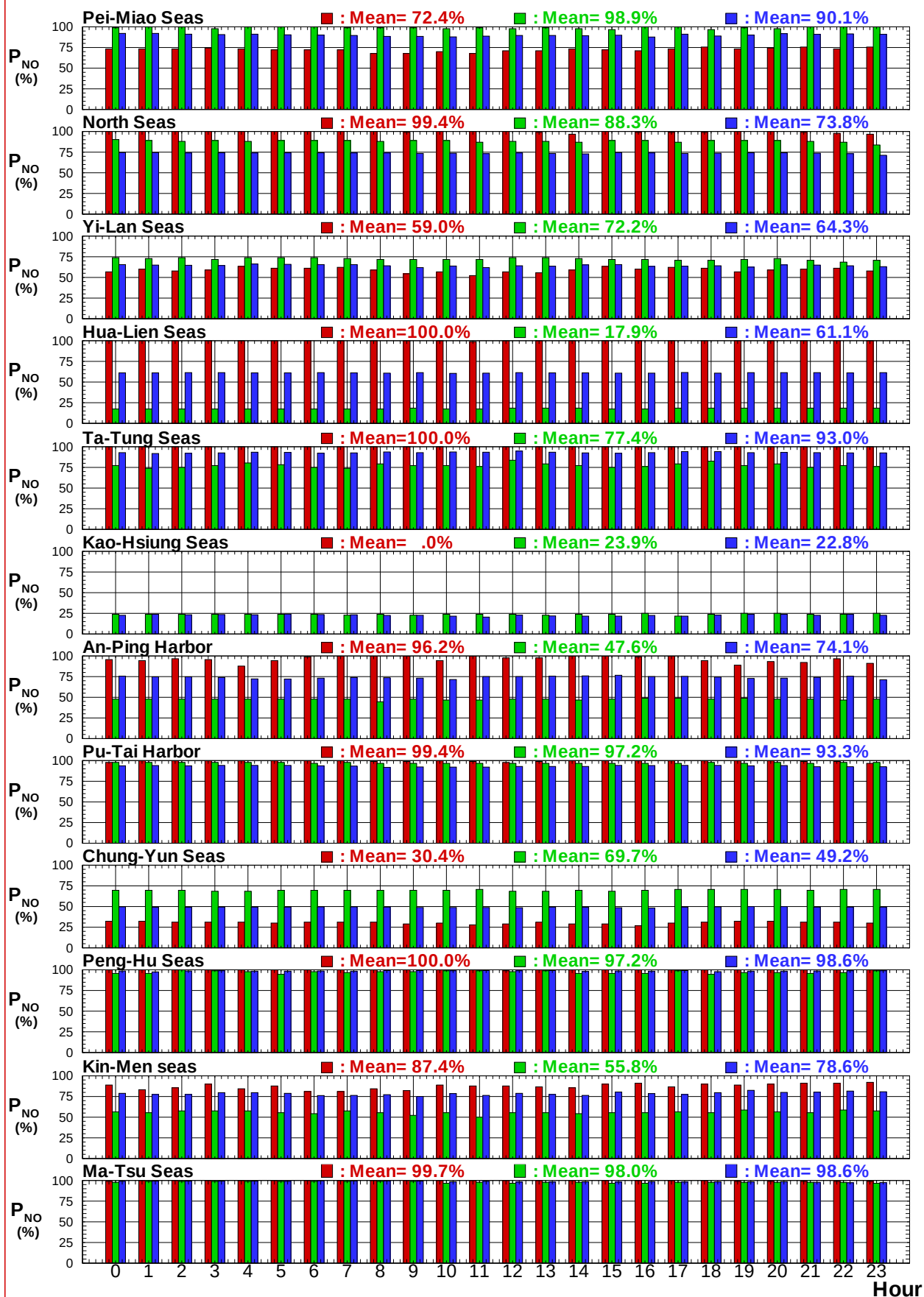
圖7.4b 2018年12港域冬, 夏及整年主要測站逐時蒐集率比較圖
