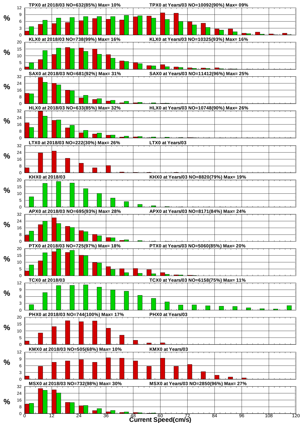
圖8.7 12港域2018年及歷年 3月流速統計方塊圖
