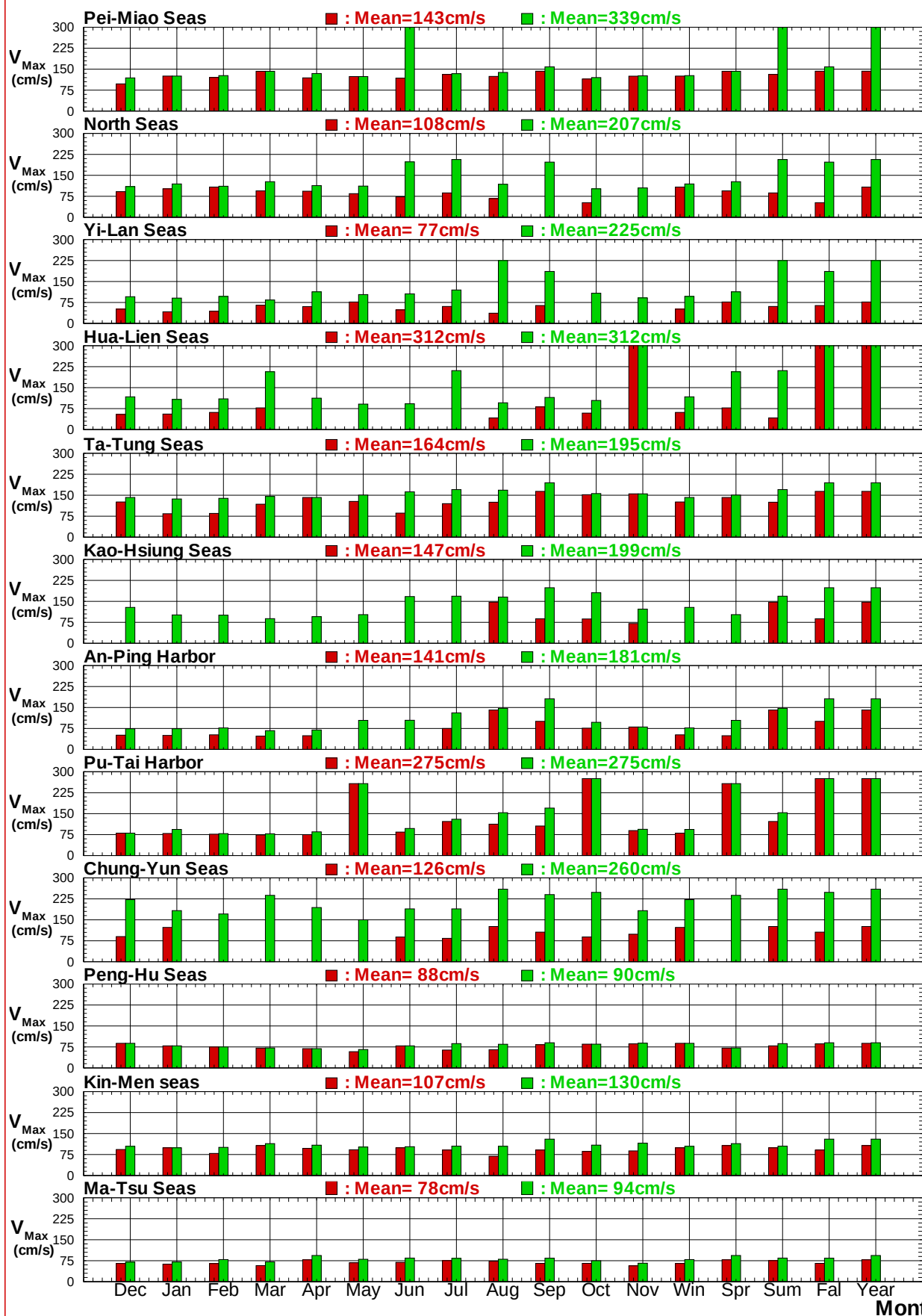
圖7.3c 2018及歷年12港域主要測站每月(季)最大流速比較圖
