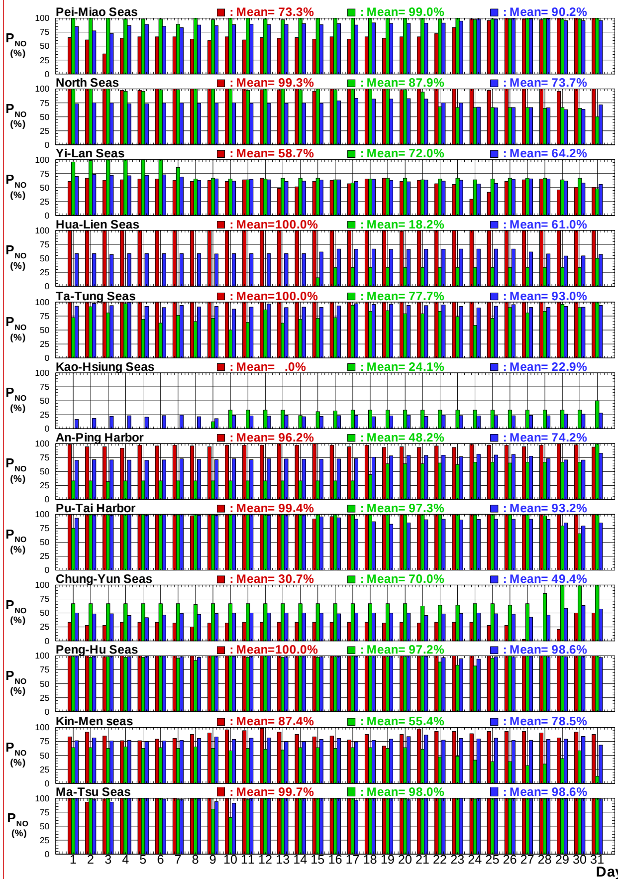
圖7.6b 2018年12港域冬, 夏及整年主要測站每日蒐集率比較圖
