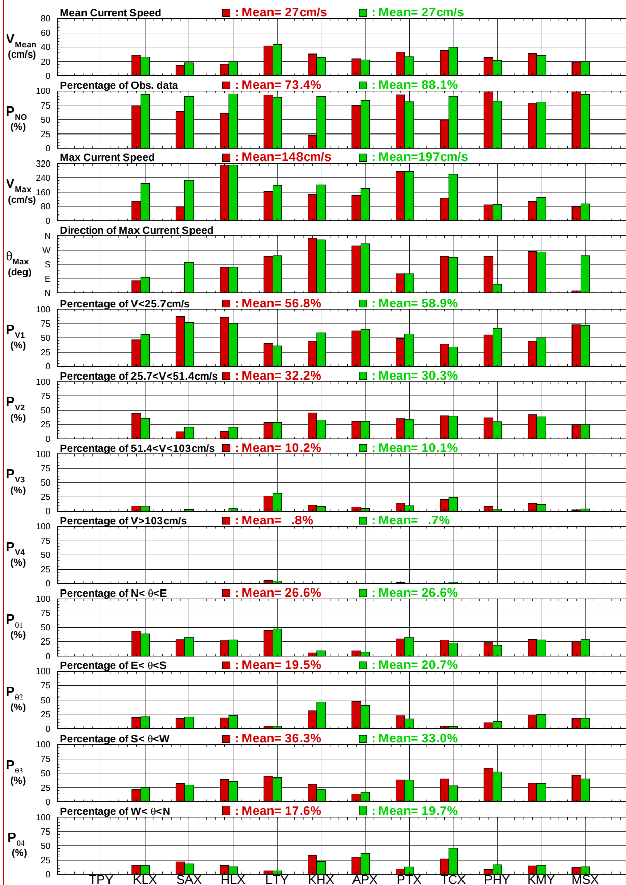
圖7.1e 12個港域2018及歷年主要測站整年流速(向)比較圖
