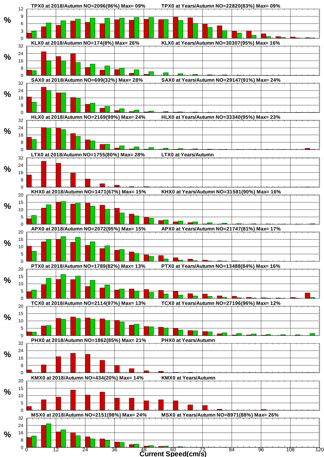
圖8.31 12港域2018年及歷年秋季流速統計方塊圖
