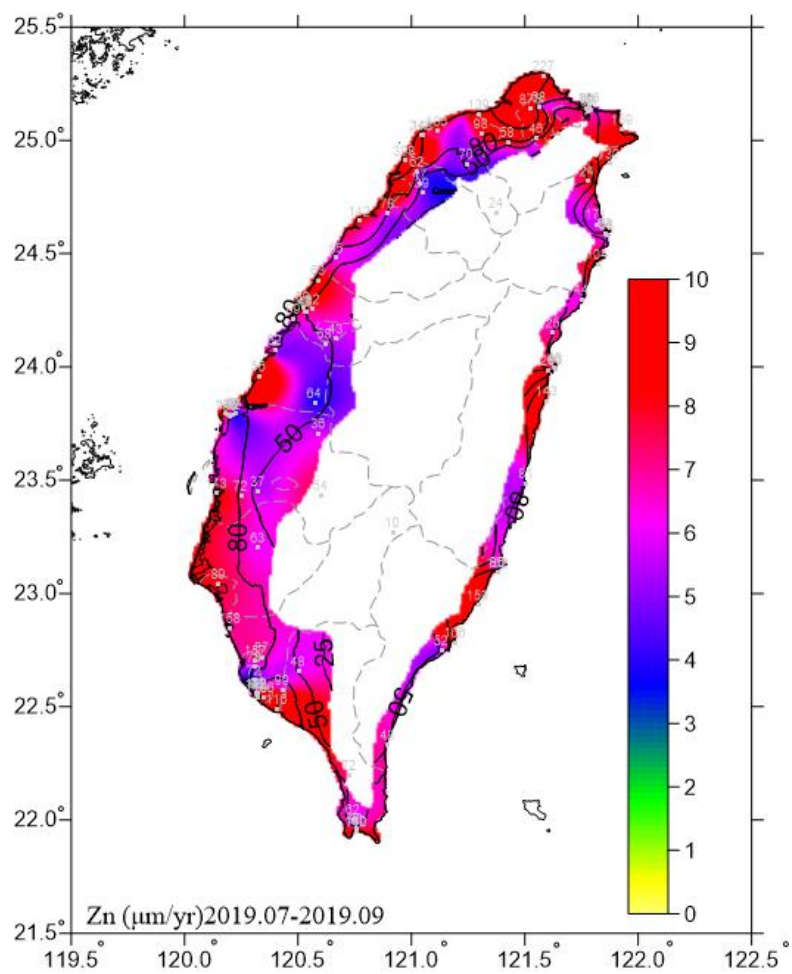
圖 6.15 2019.07-2019.09 鋅腐蝕速率圖
