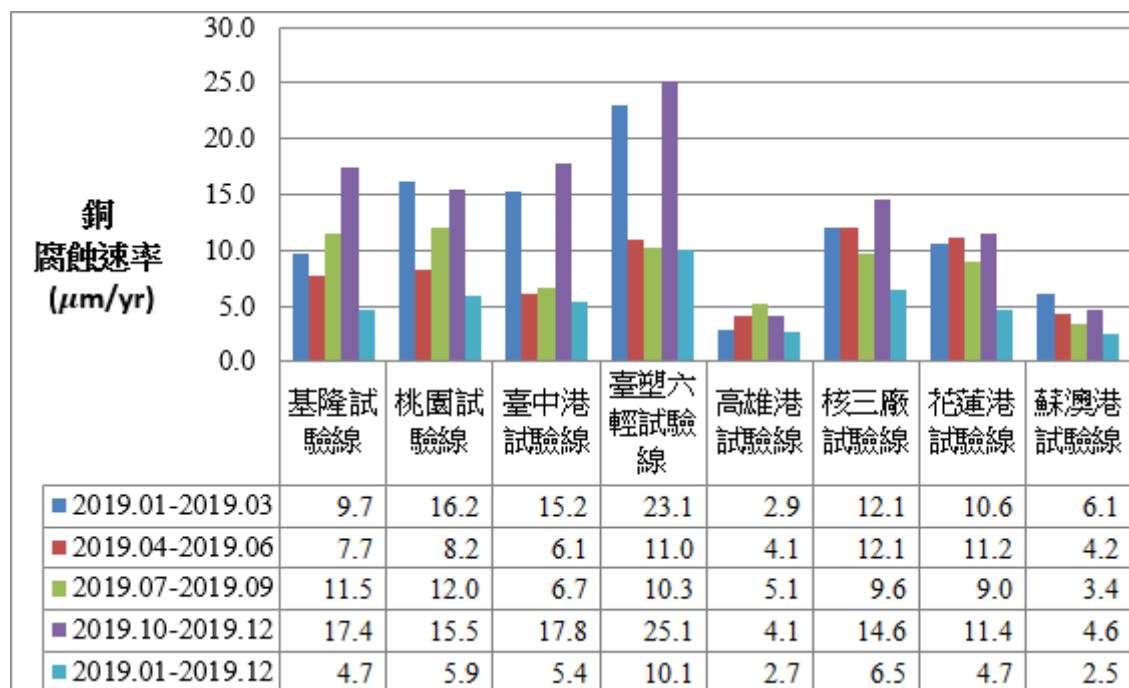
圖 6.3 垂直海岸試驗線銅腐蝕速率比較圖
