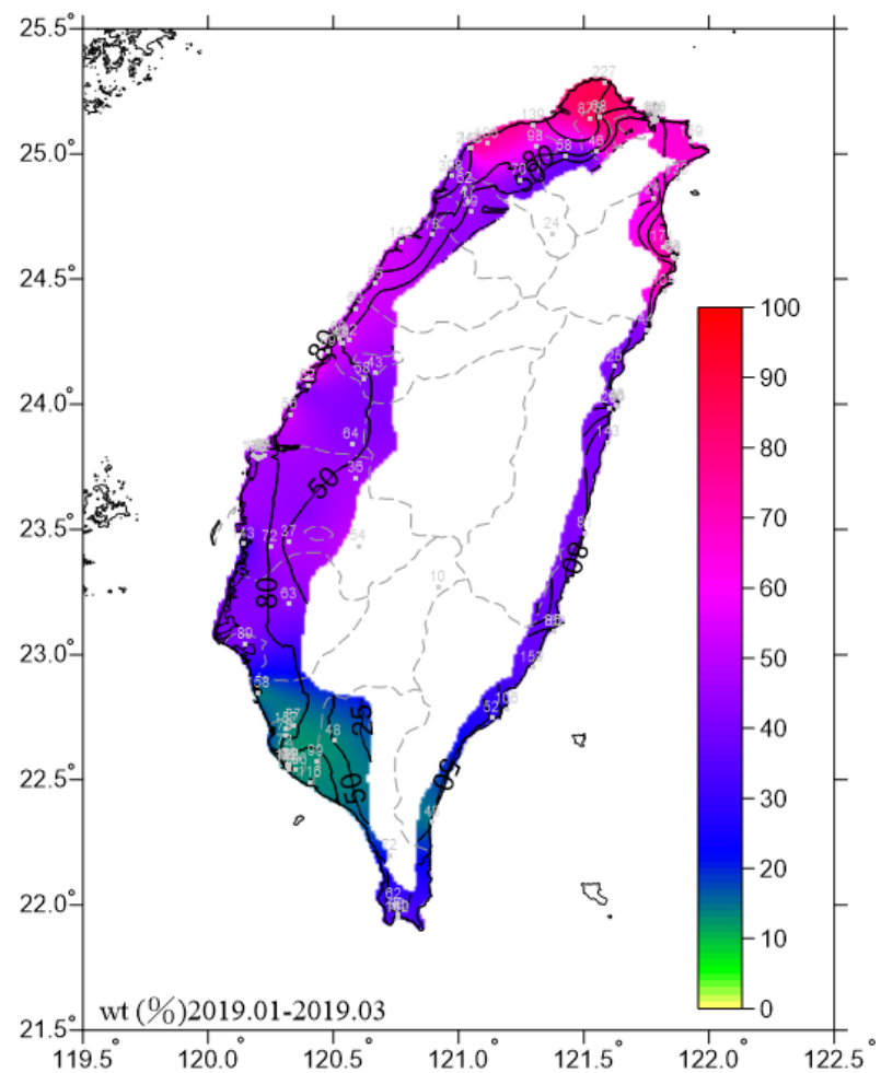
圖 3.1 2019.01-2019.03 濕潤時間圖
