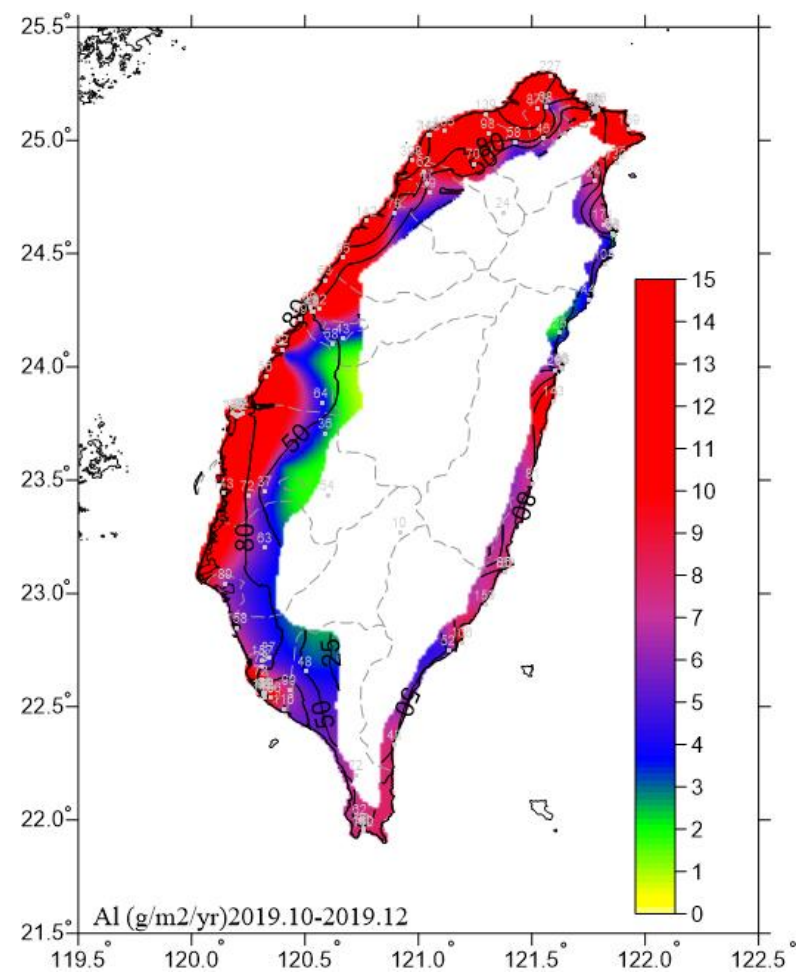
圖 6.24 2019.10-2019.12 鋁腐蝕速率圖
