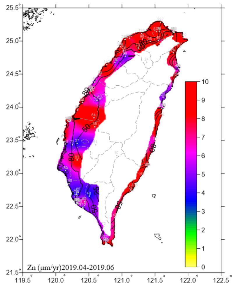
圖 6.14 2019.04-2019.06 鋅腐蝕速率圖
