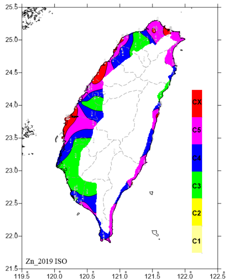
圖 6.30 2019 鋅年腐蝕速率 ISO 分類圖
