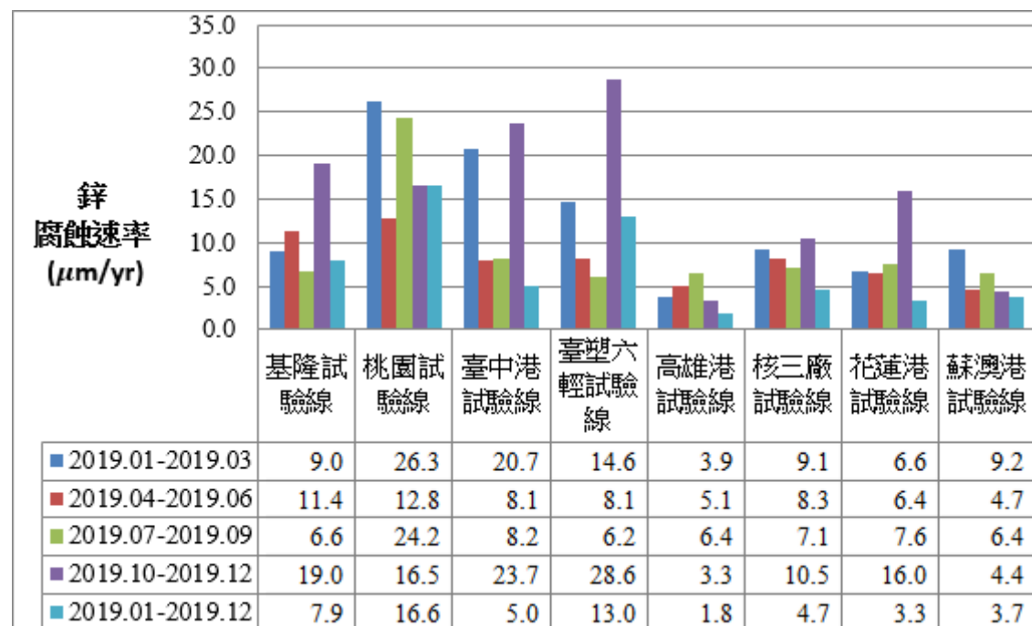
圖 6.2 垂直海岸試驗線鋅腐蝕速率比較圖
