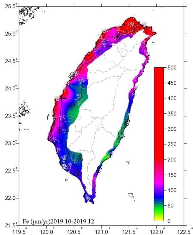
圖 6.12 2019.10-2019.12 碳鋼腐蝕速率圖
