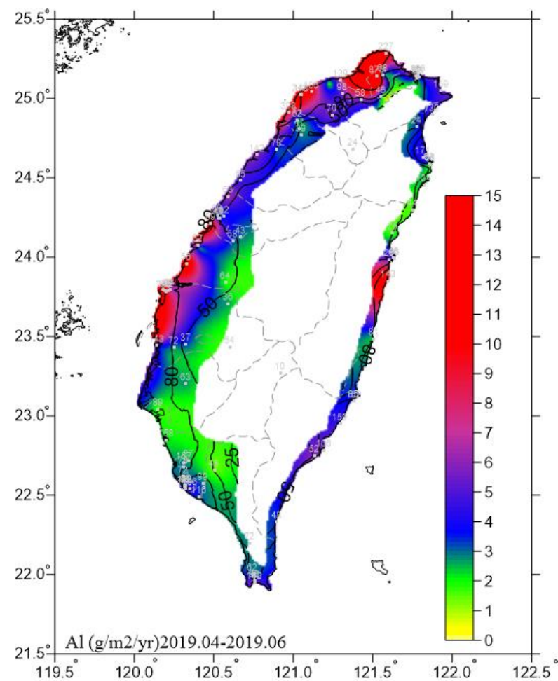
圖 6.22 2019.04-2019.06 鋁腐蝕速率圖
