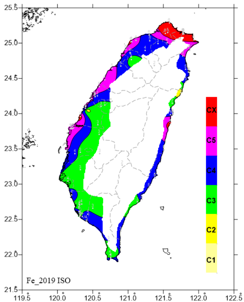
圖 6.29 2019 碳鋼年腐蝕速率 ISO 分類圖
