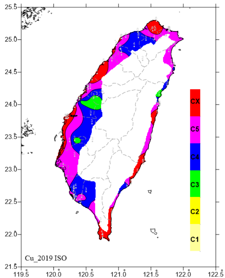
圖 6.31 2019 銅年腐蝕速率 ISO 分類圖
