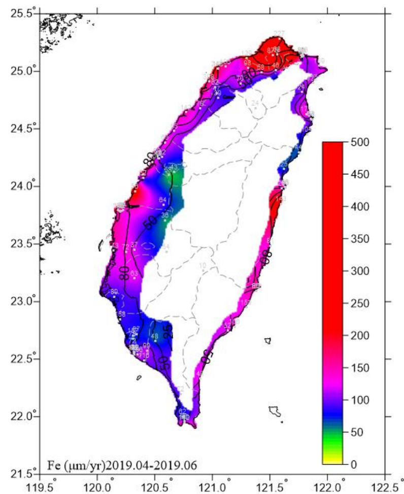
圖 6.10 2019.04-2019.06 碳鋼腐蝕速率圖
