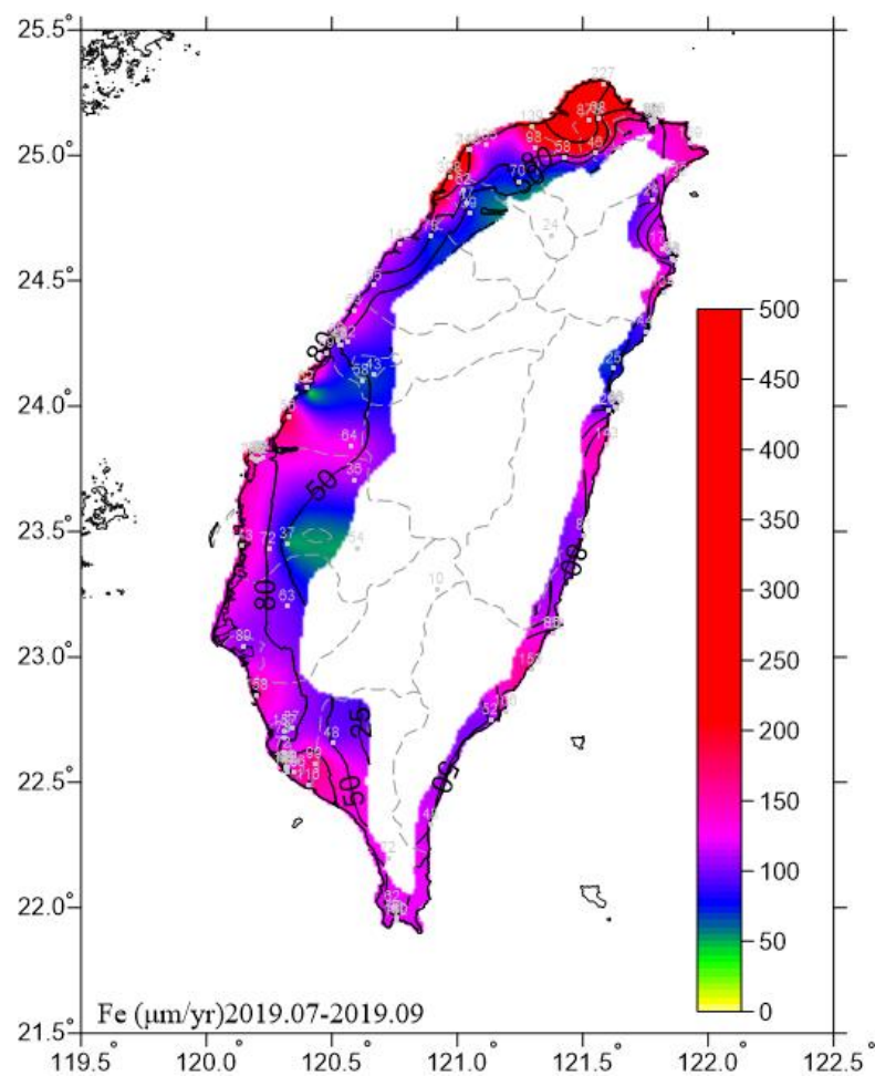
圖 6.11 2019.07-2019.09 碳鋼腐蝕速率圖
