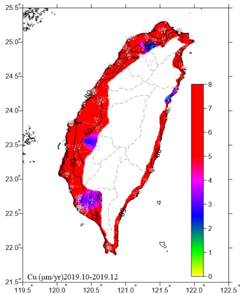
圖 6.20 2019.10-2019.12 銅腐蝕速率圖
