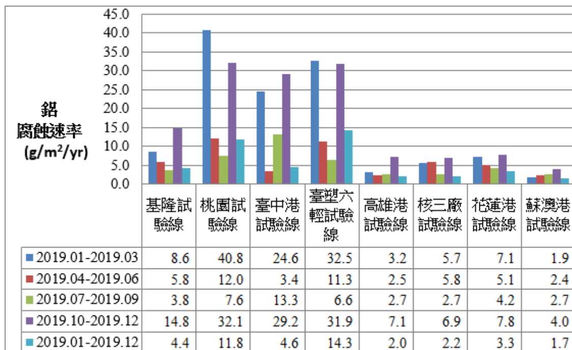
圖 6.4 垂直海岸試驗線鋁腐蝕速率比較圖
