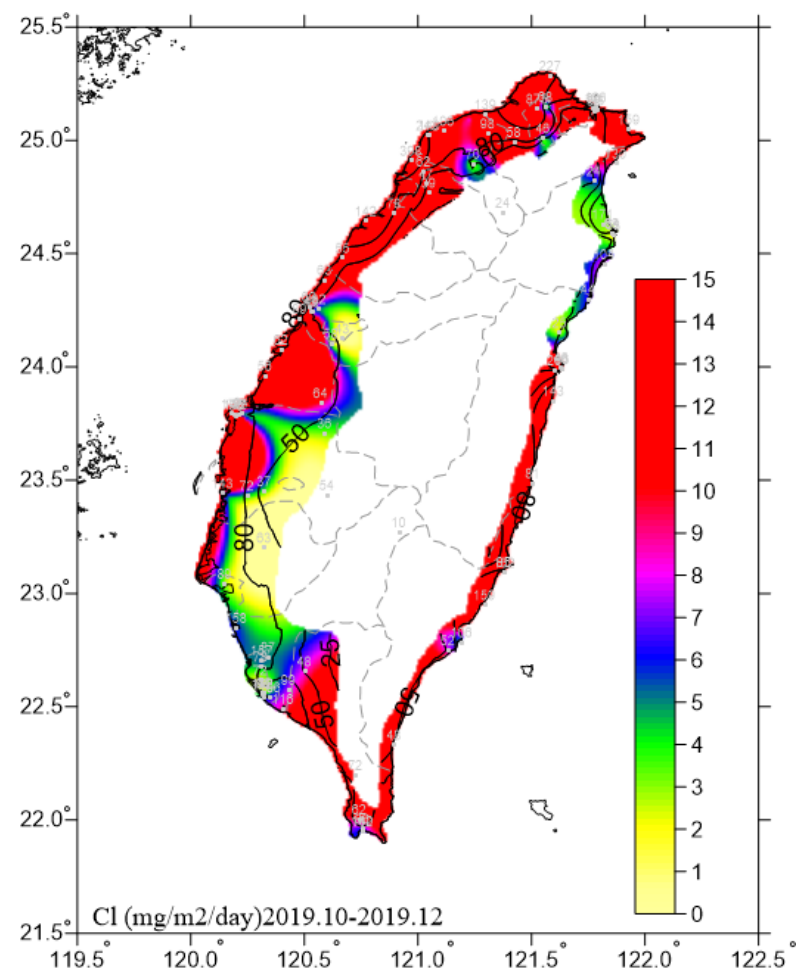
圖 4.4 2019.10-2019.12 氯鹽沉積速率圖
