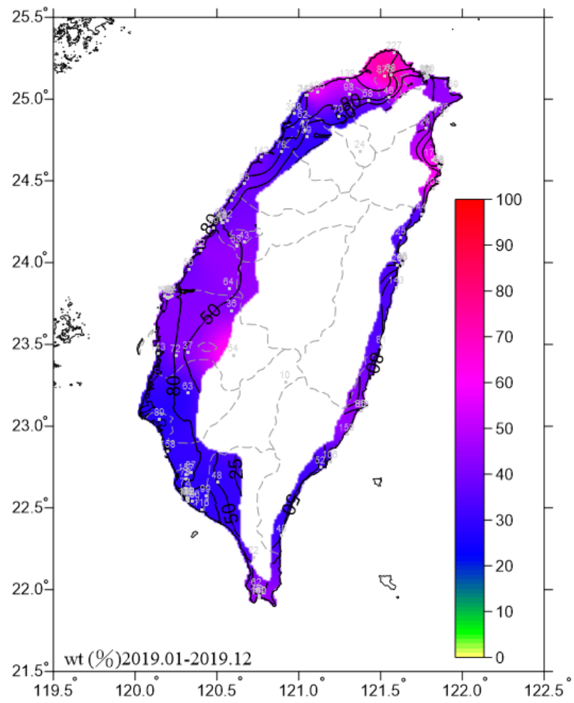
圖 3.5 2019 一年期濕潤時間圖
