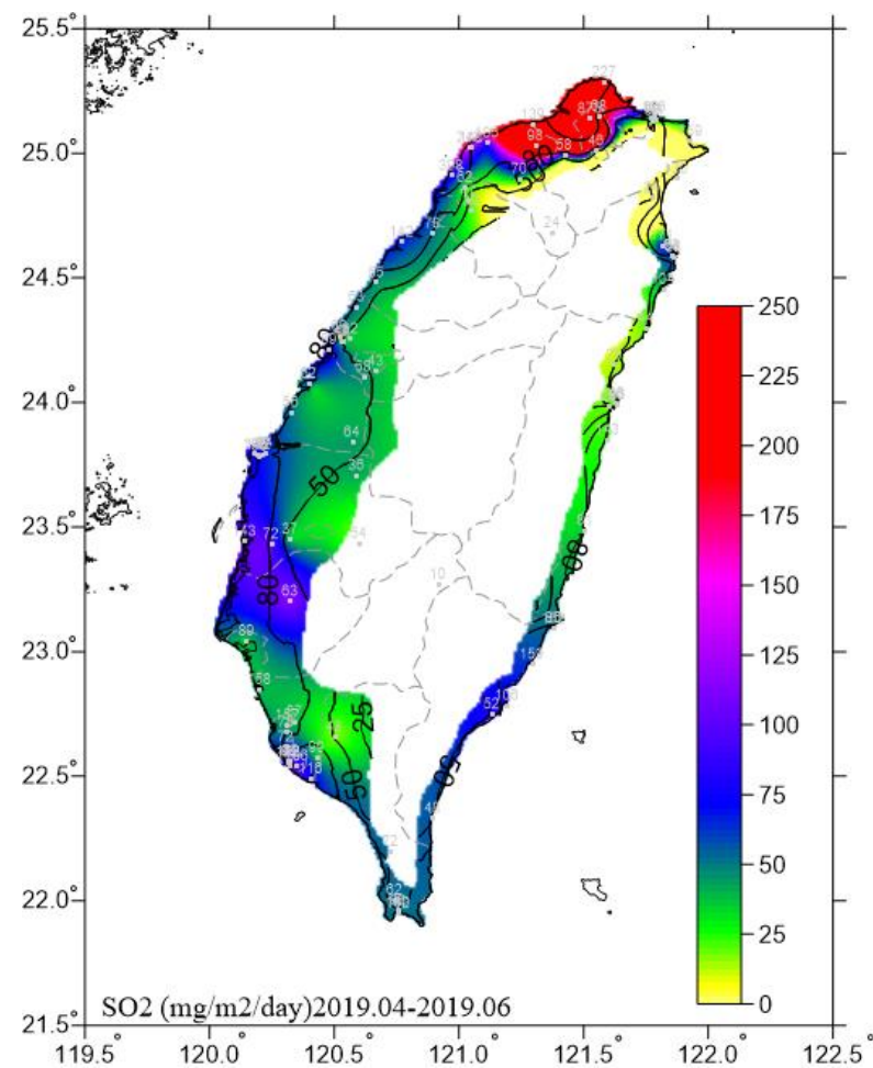
圖 5.2 2019.04-2019.06 二氧化硫沉積速率圖
