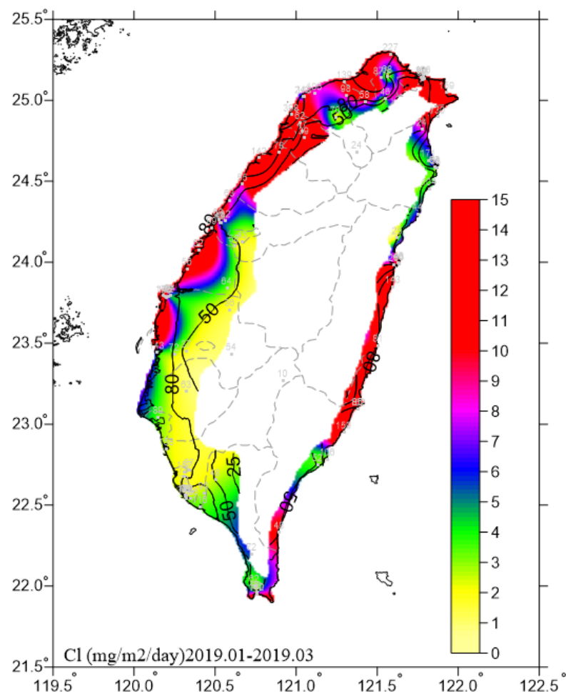
圖 4.1 2019.01-2019.03 氯鹽沉積速率圖
