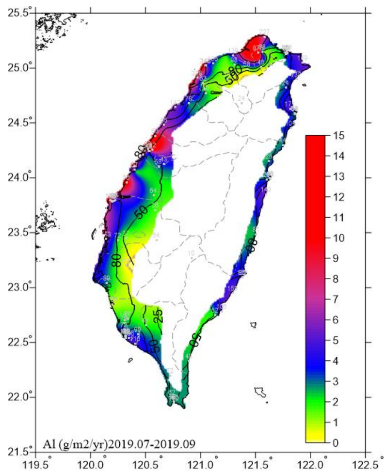
圖 6.23 2019.07-2019.09 鋁腐蝕速率圖
