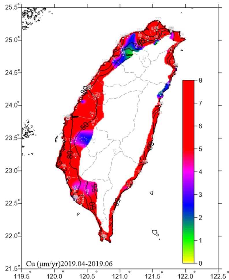
圖 6.18 2019.04-2019.06 銅腐蝕速率圖
