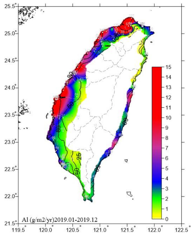
圖 6.28 2019 一年期鋁腐蝕速率
