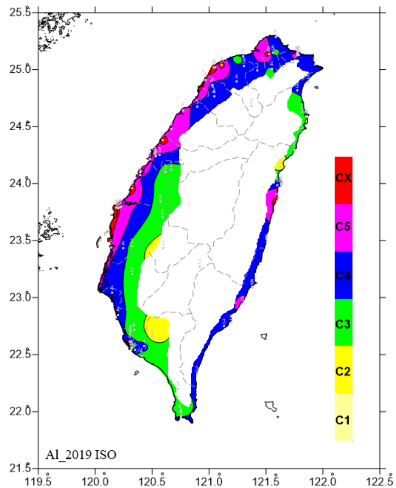
圖 6.32 2019 鋁年腐蝕速率 ISO 分類圖
