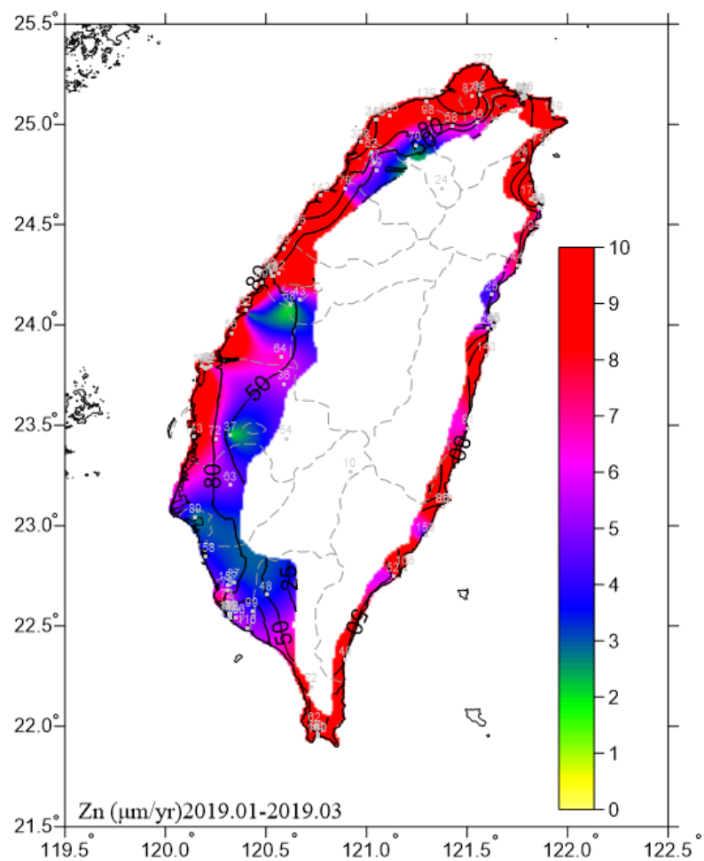
圖 6.13 2019.01-2019.03 鋅腐蝕速率圖
