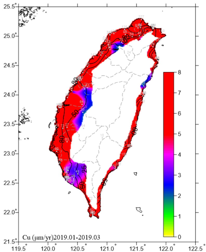
圖 6.17 2019.01-2019.03 銅腐蝕速率圖
