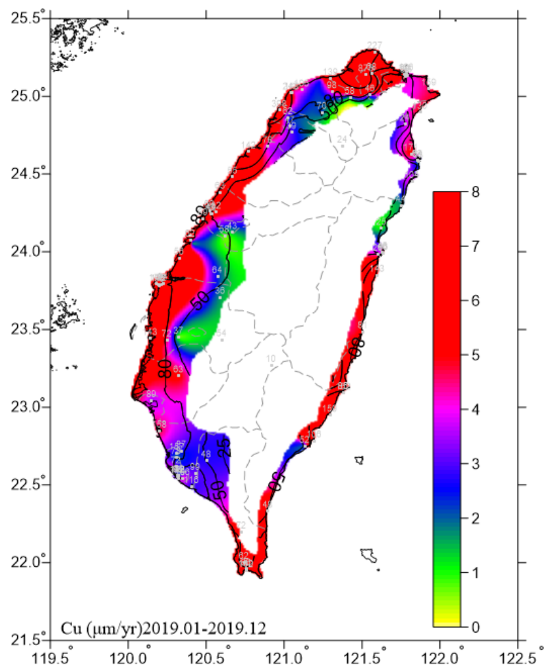
圖 6.27 2019 一年期銅腐蝕速率
