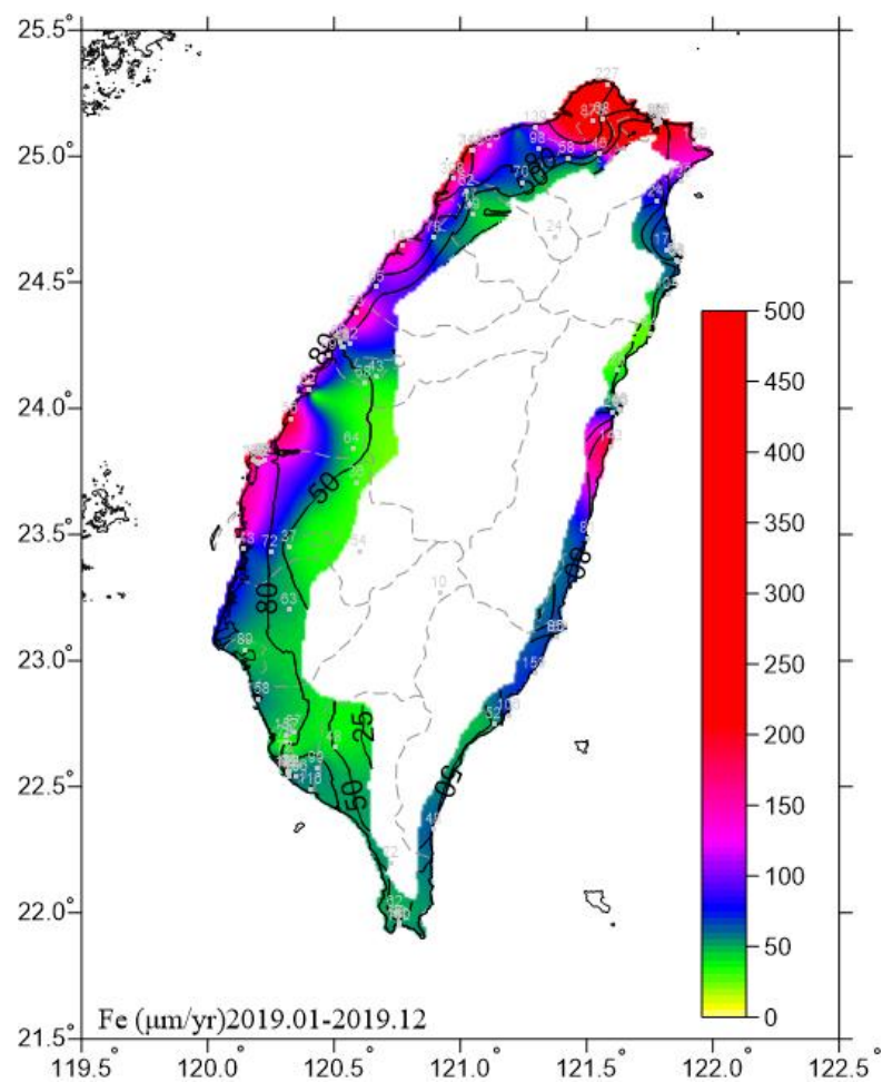
圖 6.25 2019 一年期碳鋼腐蝕速率
