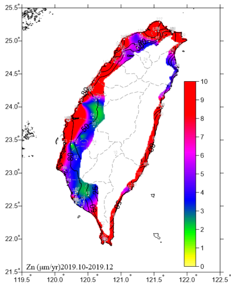
圖 6.16 2019.10-2019.12 鋅腐蝕速率圖
