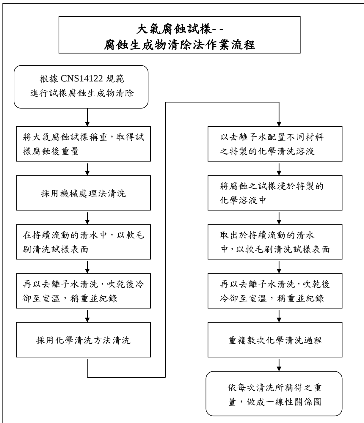
圖 1.6 腐蝕生成物清除法作業流程
