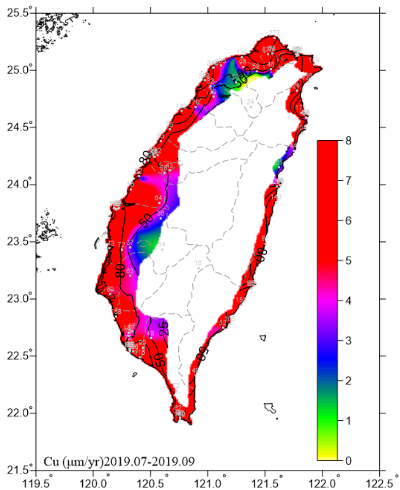
圖 6.19 2019.07-2019.09 銅腐蝕速率圖
