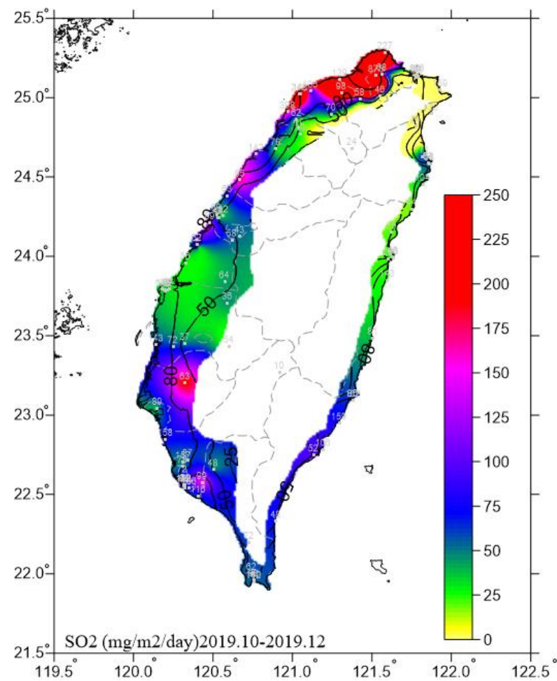
圖 5.4 2019.10-2019.12 二氧化硫沉積速率圖
