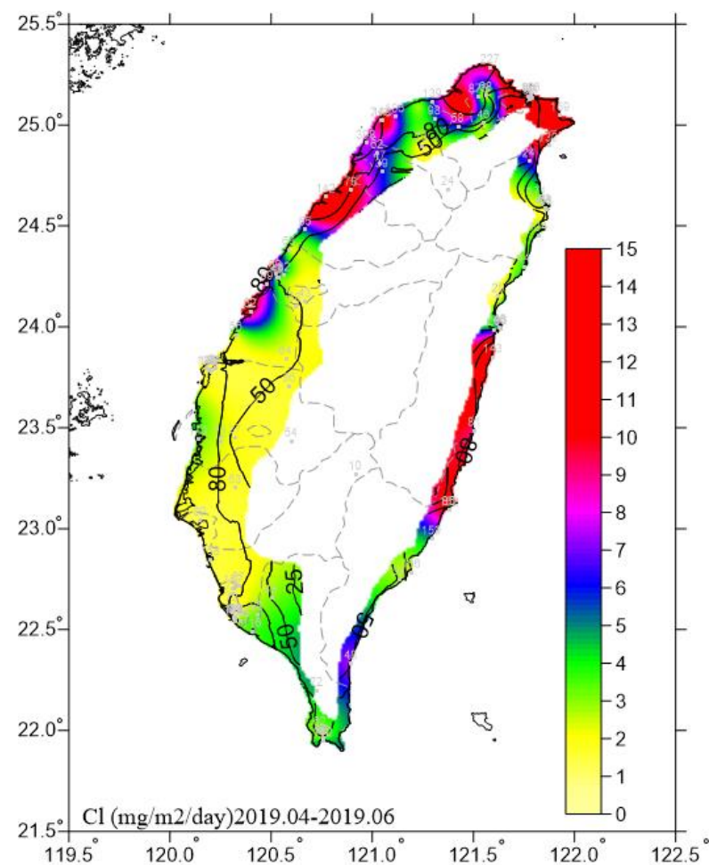
圖 4.2 2019.04-2019.06 氯鹽沉積速率圖
