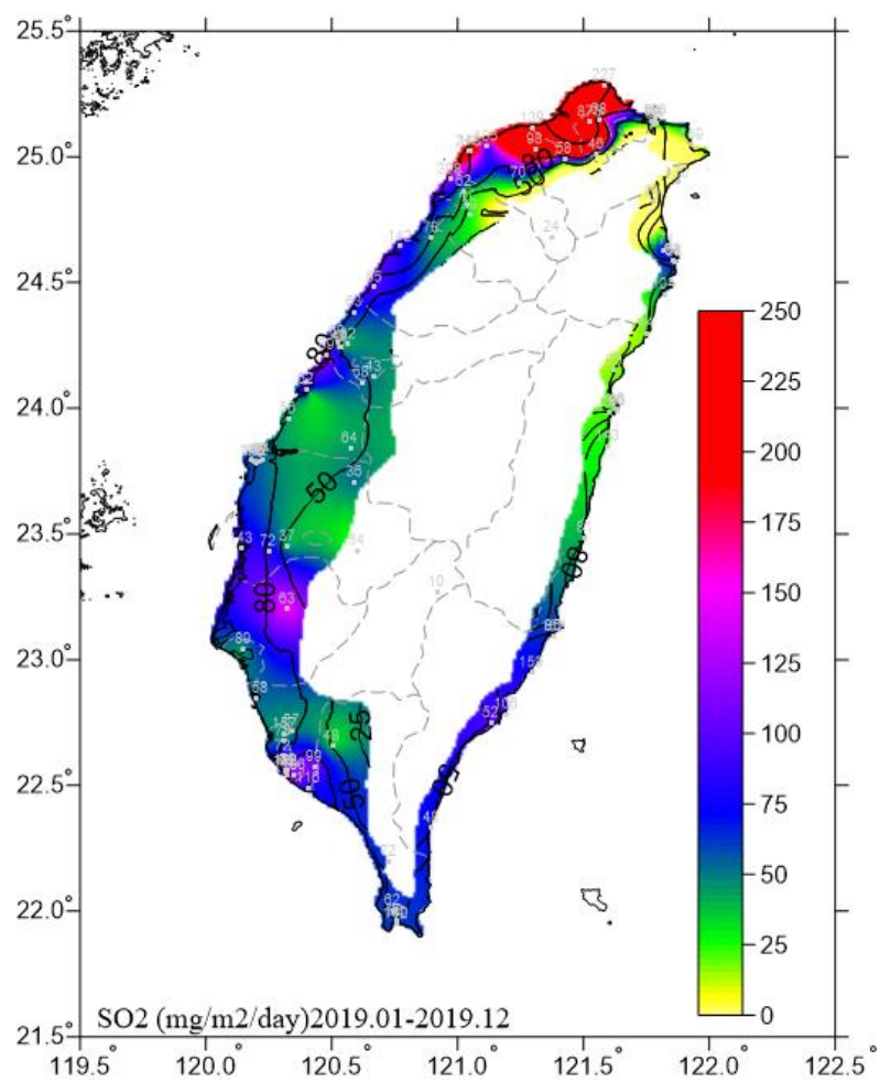
圖 5.5 2019 二氧化硫沉積速率圖
