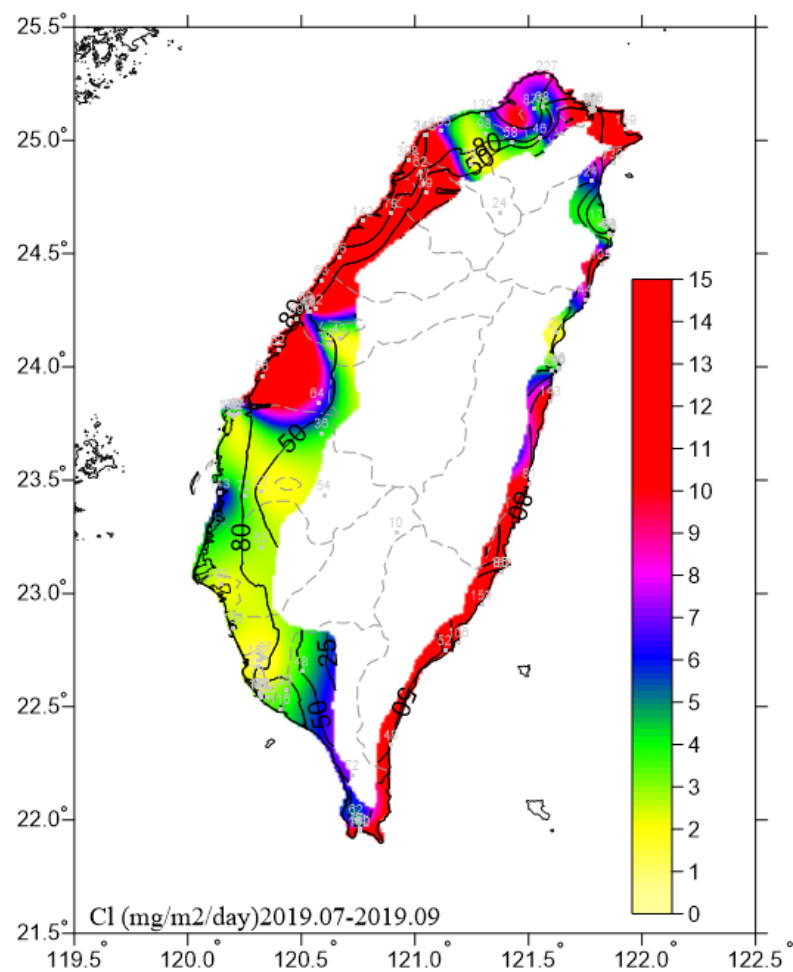
圖 4.3 2019.07-2019.09 氯鹽沉積速率圖
