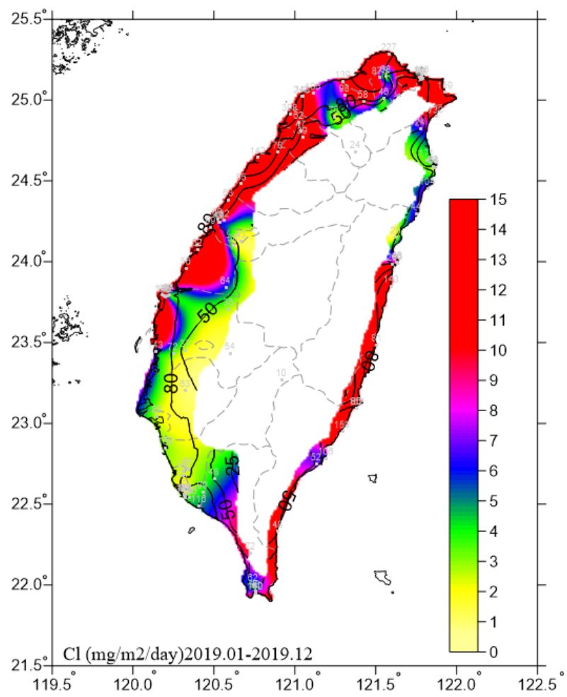
圖 4.5 2019 一年期氯鹽沉積速率圖
