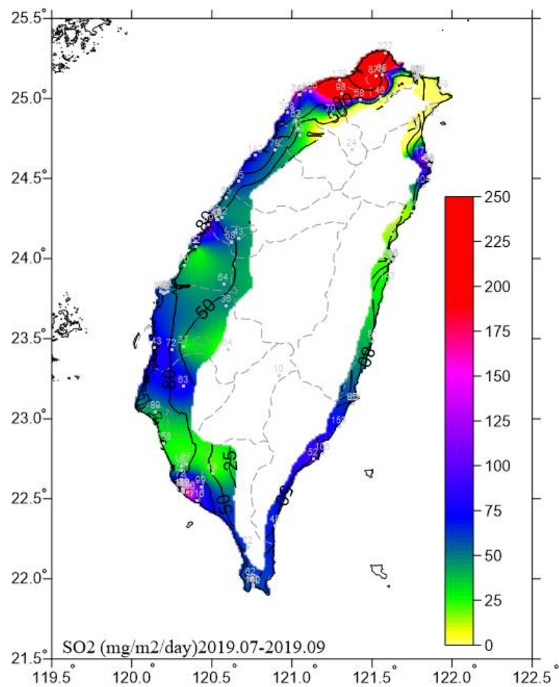
圖 5.3 2019.07-2019.09 二氧化硫沉積速率圖
