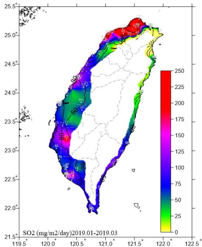
圖 5.1 2019.01-2019.03 二氧化硫沉積速率圖
