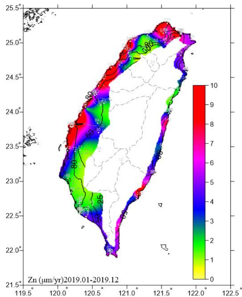
圖 6.26 2019 一年期鋅腐蝕速率
