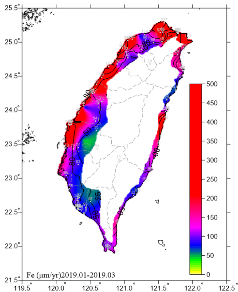
圖 6.9 2019.01-2019.03 碳鋼腐蝕速率圖
