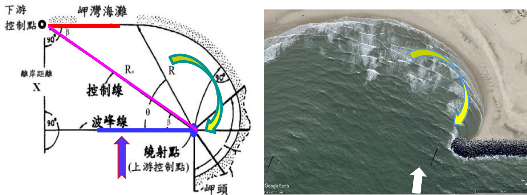
圖 4-38 岬頭後因折、繞射波浪碎波之直接沖刷環流作用而造成繫岸沙洲型態之岬灣海灘重塑
