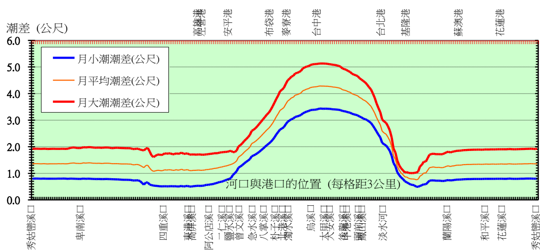
圖 2-19 臺灣環島沿岸各主要河川河口與各重要工商港口位置之月大、小潮及月平均潮差分布
