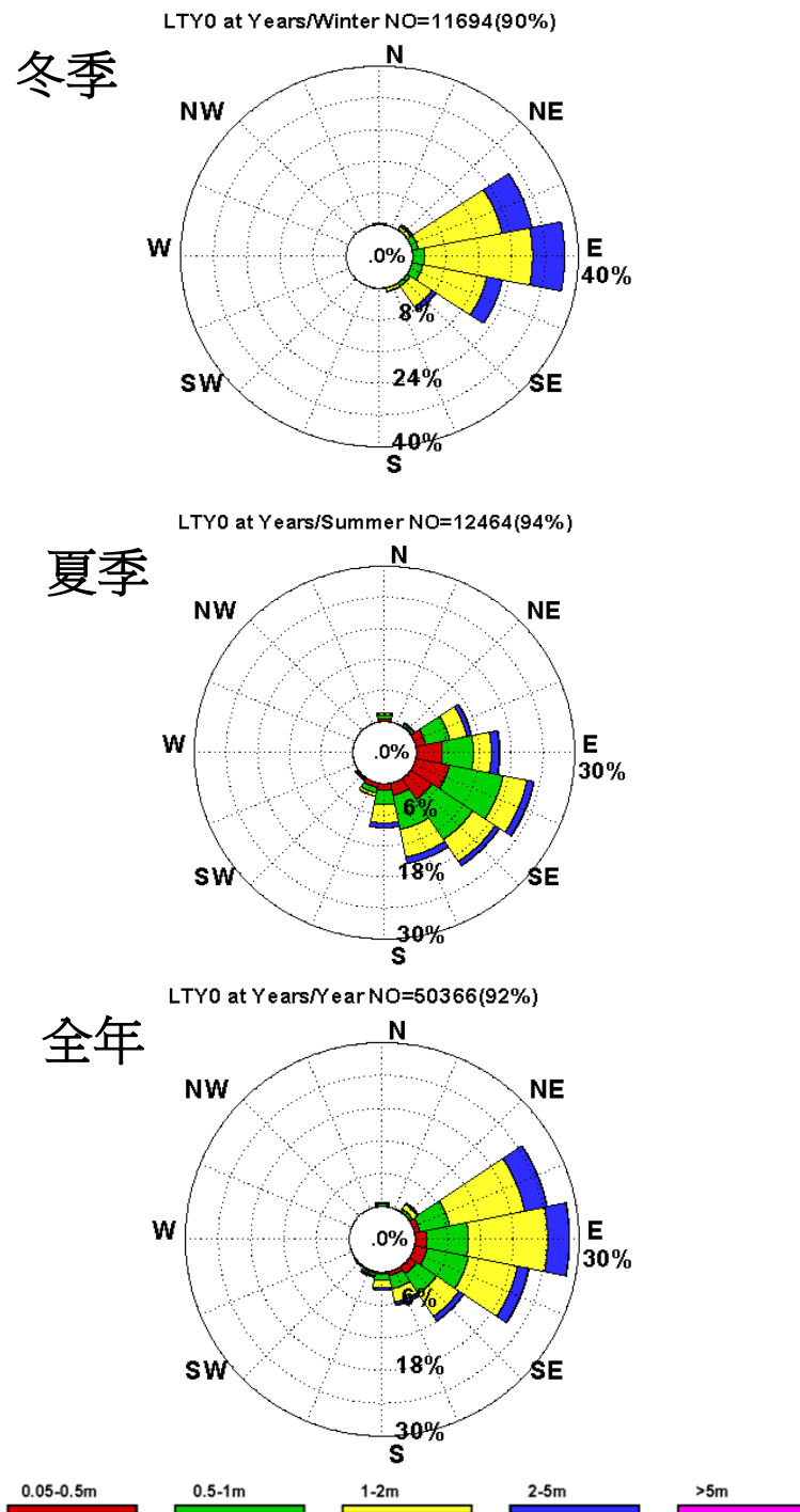
圖 4-46 臺東海域概約自 2000 年起至 2016 年止冬季(上)、夏季(中)及全年(下)之觀測波浪玫瑰圖
