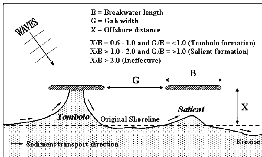
圖 4-29 近岸海灘設置離岸堤群之配置定義及於堤後因波浪直接沖刷作用所造成海灘之沖淤重塑型態
