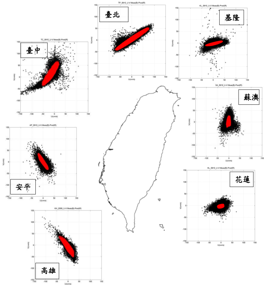
圖 2-21 臺灣七大商港港口外廓海域 2009 年至 2010 年實測海流(黑)與天文潮流(紅)之近岸流速散佈圖比較
