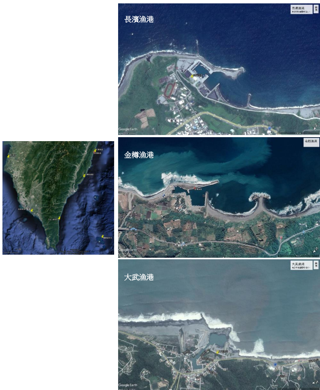
圖 4-45(續) 臺東海岸面對冬、夏季主要波浪入射方向之長濱(右上)、金樽(右中)及大武(右下)漁港既有複合離岸堤及突堤型態之港口配置及與港口毗鄰海岸之防護設施
