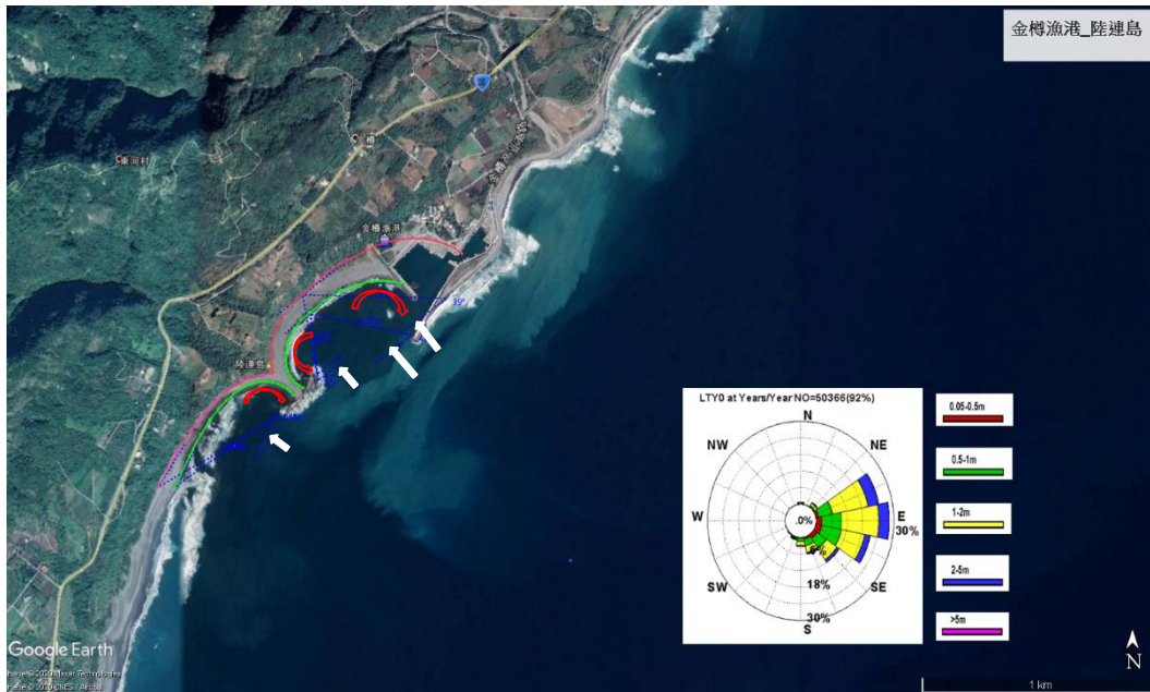
金樽漁港_陸連島_岬頭灘線_港口擴建後現況_波浪玫瑰圖_20190302_1. jpg
