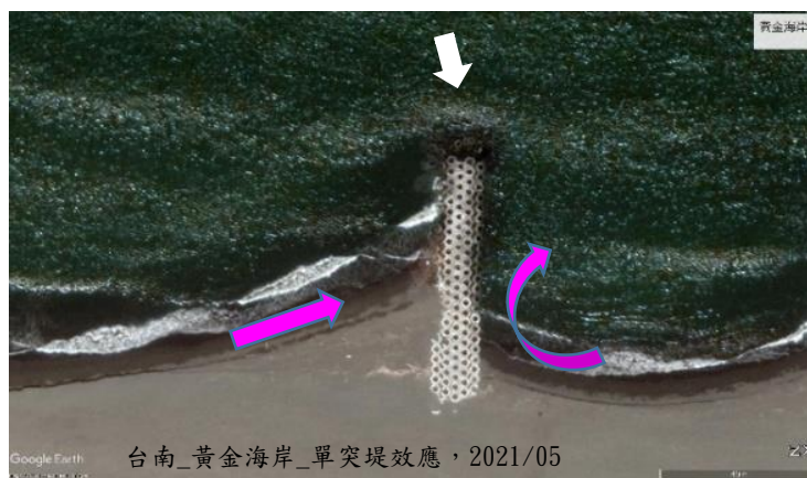
圖 4-19 在近岸海灘設置突堤後因受波浪碎波之冲刷流作用所衍生迎向波浪上游側漂沙淤積而下游側沖蝕之「突堤效應」
