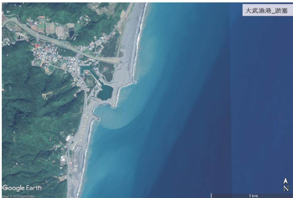
大武漁港_淤塞_Google earth_20190321_現況
