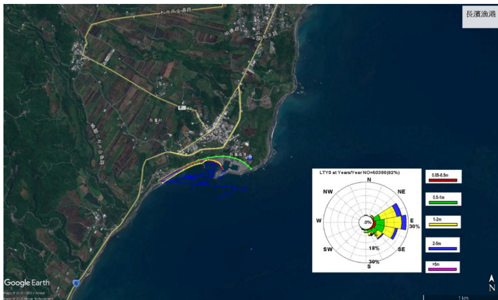
長濱漁港_海岸_岬灣海灘_現況_波浪玫瑰圖_20190328.tiff
