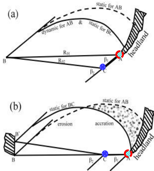
圖 4-37 從輸沙不平衡會造成灘線侵淤之觀點探討靜態及動態岬灣海灘之穩定性
