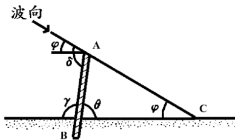
圖 4-18 灘線及突堤配置與主要波向之相關性
