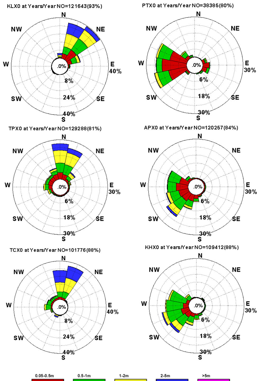
圖 2-14 臺灣西北部基隆(左上)、臺北(左中)、臺中(左下)及臺灣西南部布袋(右上)、安平(右中)、高雄(右下)海域自 2000 年起至 2016 年止歷年觀測全年波浪玫瑰圖
