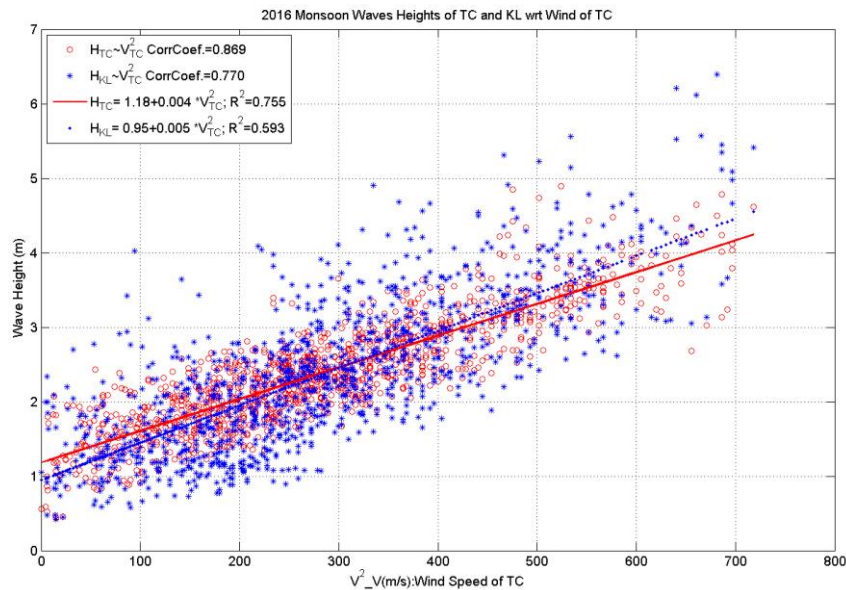
圖 2-6 冬季季風期間臺灣西部海岸臺中港(紅)及北部海岸基隆港(藍)之季風波浪示性波高與臺中港風速二次方之關聯圖
