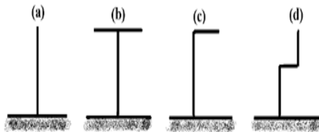
圖 4-17 突堤的平面型式(a)突堤型(b)T 型(c)倒 L 型(d)側 Z 型
