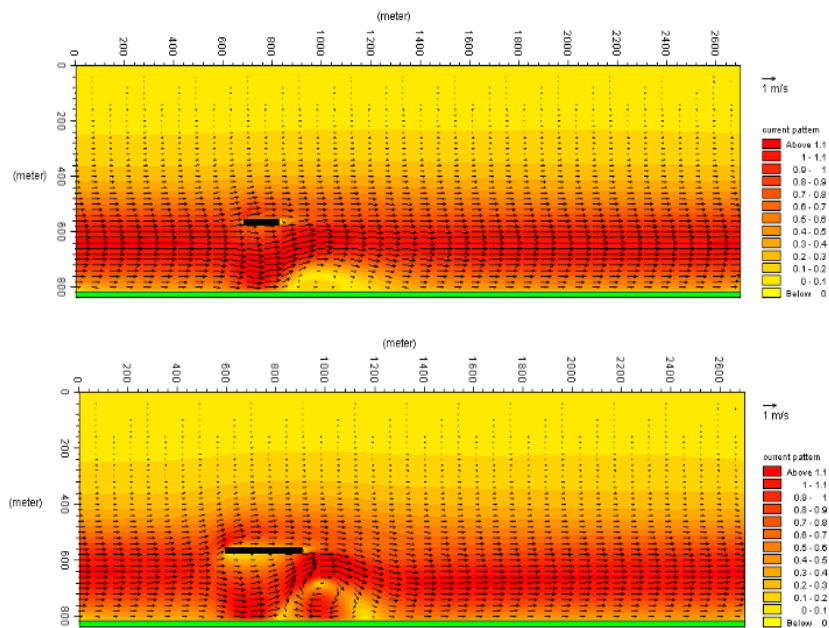
圖 4-28 均勻坡度海灘上受波浪斜向入射之短(上)、長(下)離岸堤鄰近之近岸流場
