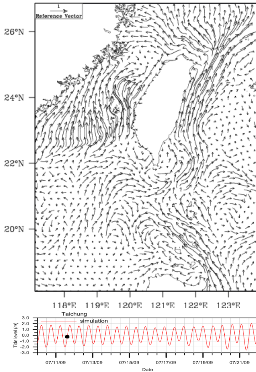
圖 2-24 臺灣海域綜合洋流與潮流效應之擬真海流流場(參考台中港漲潮期計算潮位 2009/07/11 15:00)
