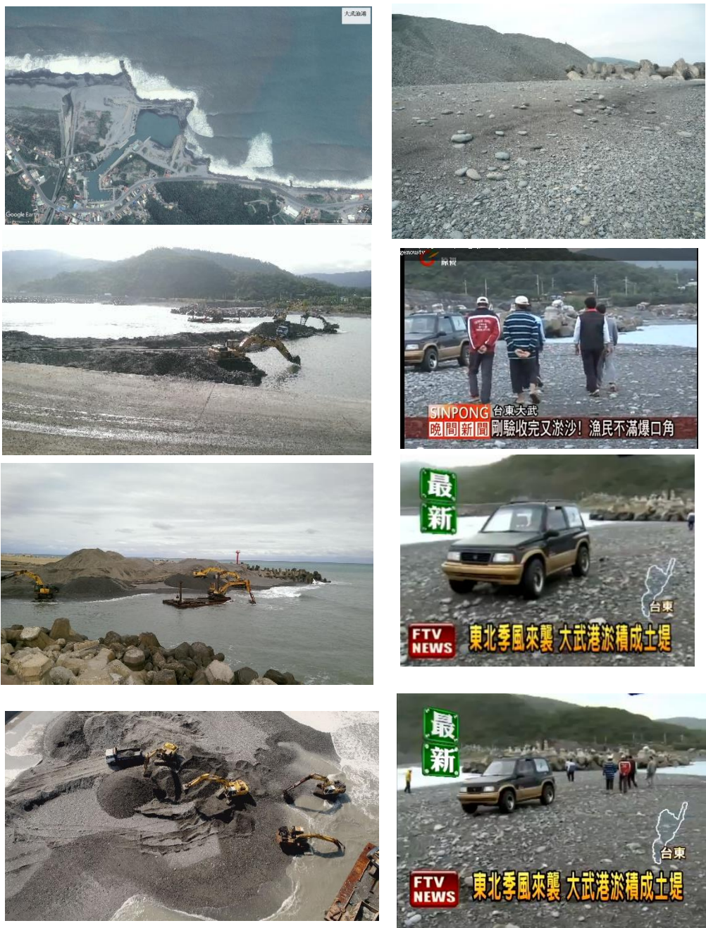
圖 4-44(續) 臺東大武漁港淤塞與清淤疏浚景況(左)及淤塞於港口航道上之大粒徑表面沉積砂石(右)
