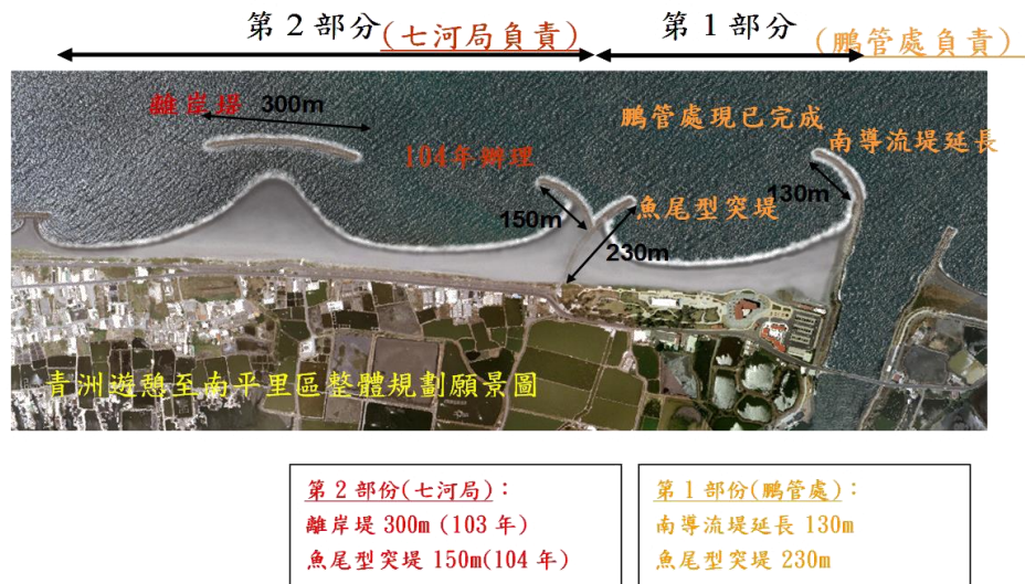
圖 4-31(續) 臺灣西南部屏東青洲遊憩區海岸環境營造整體規劃建置離岸堤與魚尾型突堤及人工岬灣等海岸防護設施後於堤後經海灘重塑之沙舌與繫岸沙洲
