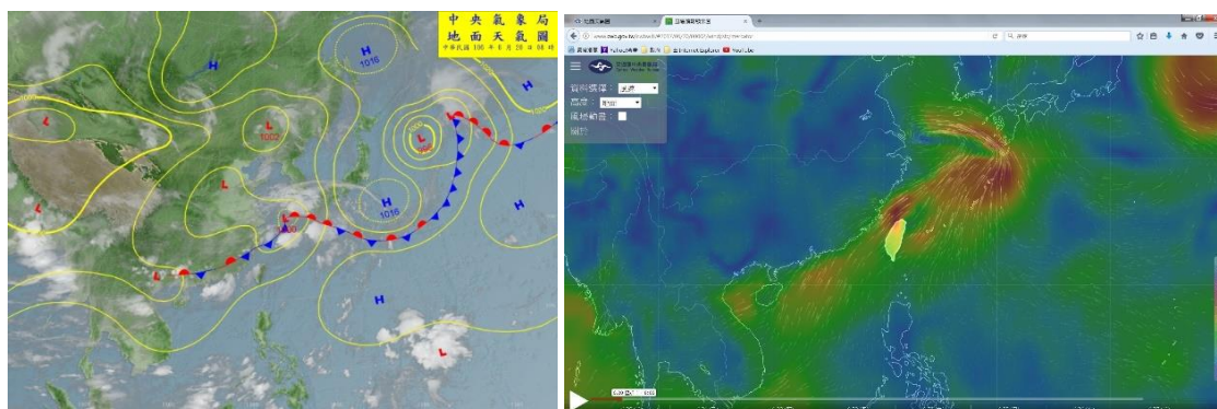
圖 2-2 臺灣海域冬季 2017/10/30 02:00 之東北季風天氣系統(左)與地面風場(右)
