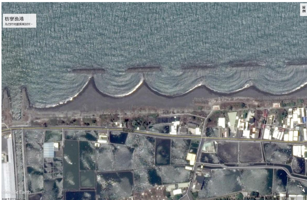
塭豐海堤_google 地圖離岸堤群 2015 平小. jpg
