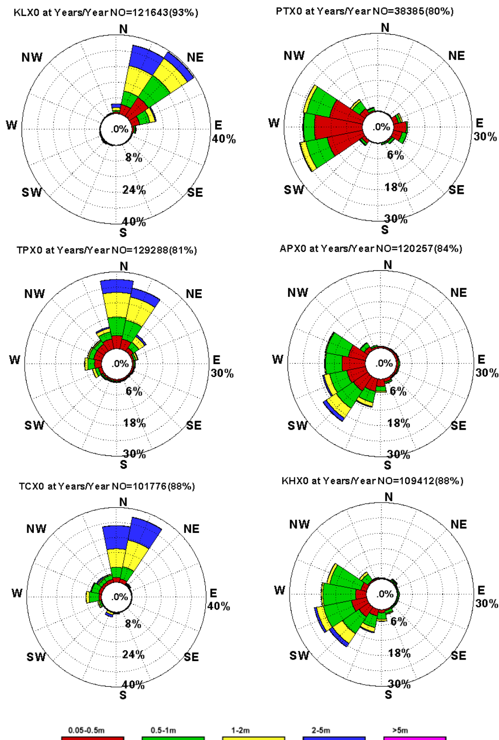
圖 4-68 臺灣西北部基隆(左上)、臺北(左中)、臺中(左下)及臺灣西南部布袋(右上)、安平(右中)、高雄(右下)海域自 2000 年起至 2016 年止歷年觀測全年波浪玫瑰圖
