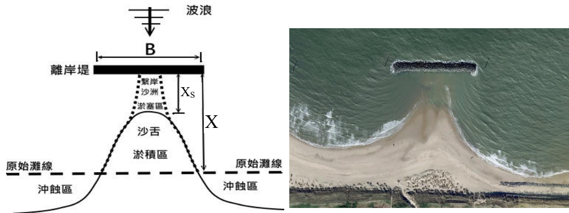
圖 4-24 近岸海灘設置離岸堤之配置定義及於堤後因波浪直接冲刷作用所造成海灘之沖淤重塑型態
