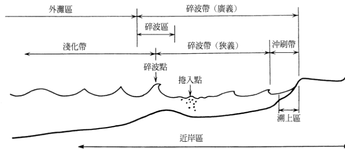
圖 1-1 近岸灘區之波浪碎波帶示意圖
