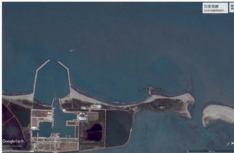
青山港汕_google 地圖 2016_突堤效應
