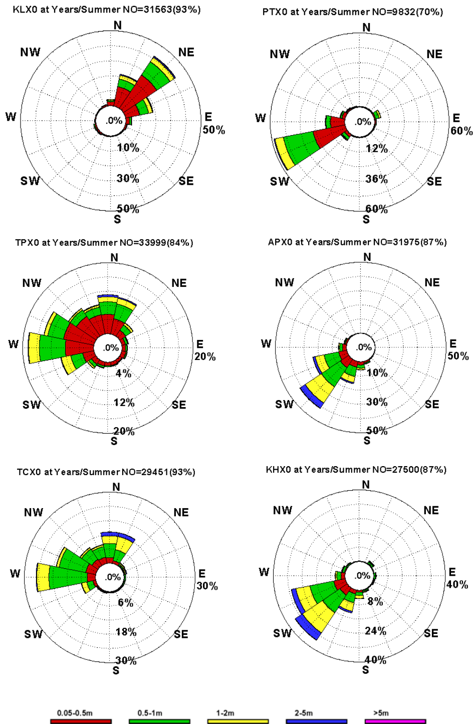
圖 2-12 臺灣西北部基隆(左上)、臺北(左中)、臺中(左下)及臺灣西南部布袋(右上)、安平(右中)、高雄(右下)海域自 2000 年起至 2016 年止歷年觀測夏季波浪玫瑰圖
