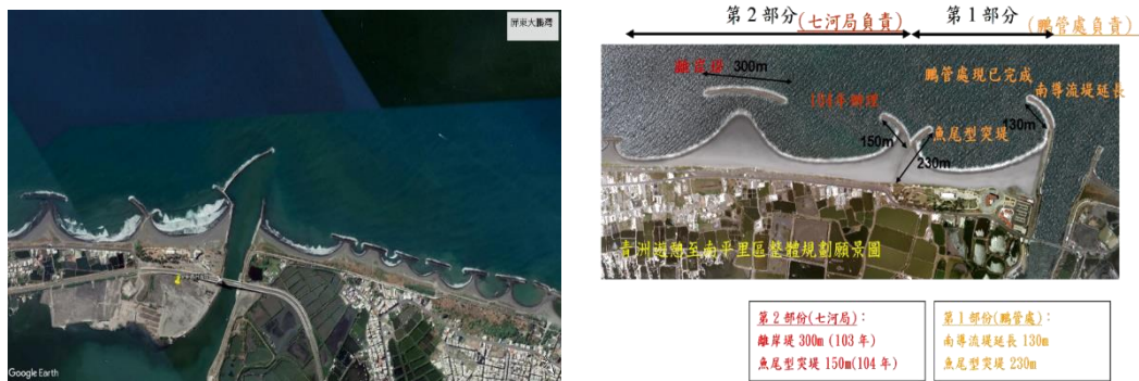
圖 4-5 臺灣環島海岸通常構建具突堤與離岸堤型態之人工防護設施
