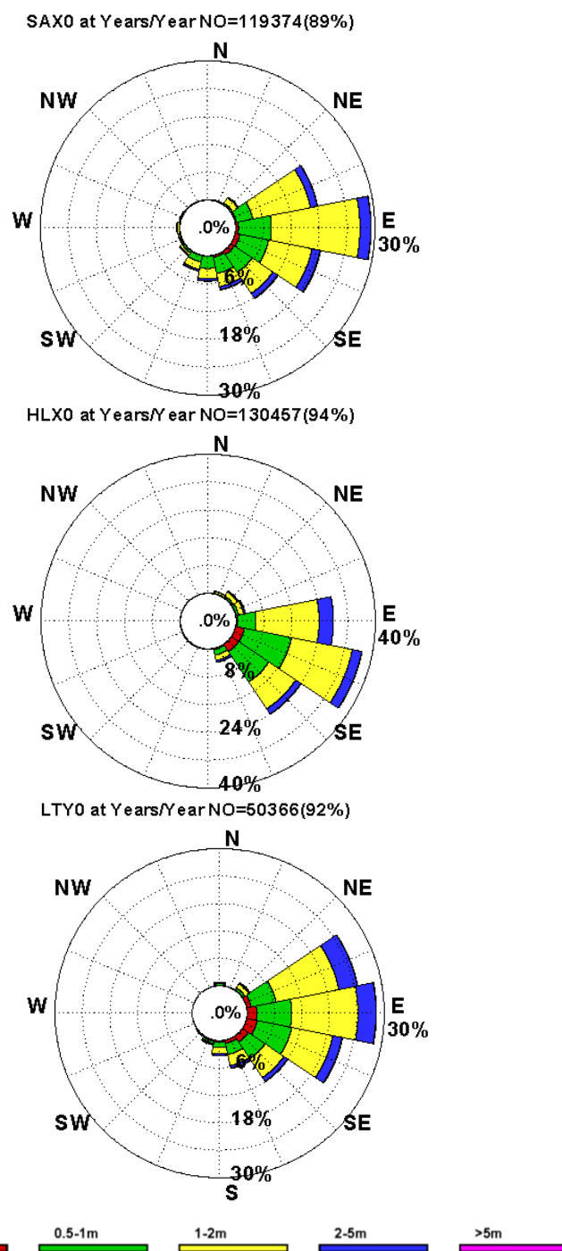
圖 2-17 臺灣東部蘇澳(上)、花蓮(中)、臺東(下)海域概約自 2000 年起至 2016 年止歷年觀測全年波浪玫瑰圖
