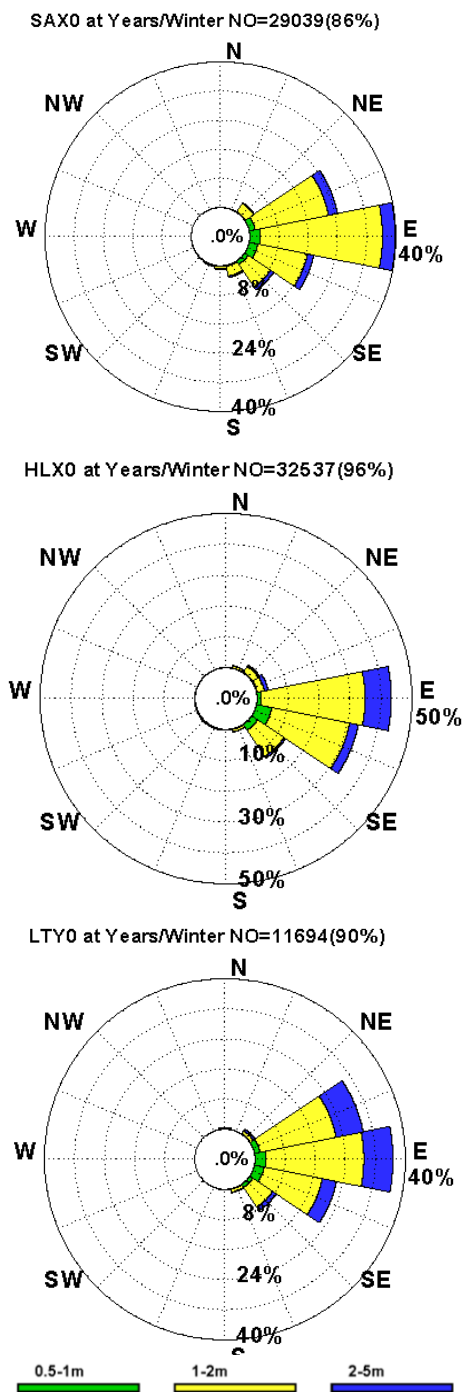
圖 2-16 臺灣東部蘇澳(上)、花蓮(中)、臺東(下)海域自 2000 年起至 2016 年止歷年觀測冬季波浪玫瑰圖
