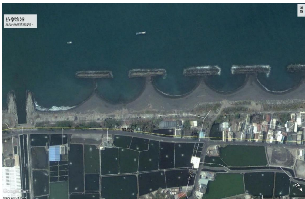
塭豐海堤_google 地圖離岸堤群 2005 平小.jpg
