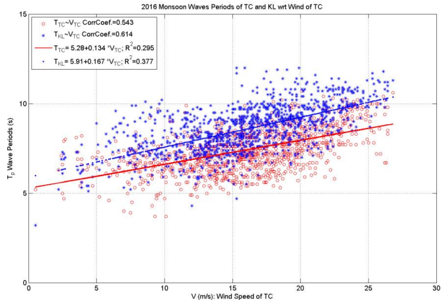
圖 2-7 冬季季風期間臺灣西部海岸臺中港(紅)及北部海岸基隆港(藍)之季風波浪尖峰週期與臺中港風速之關聯圖
