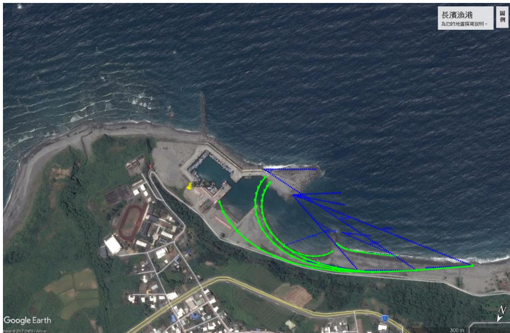
長濱漁港_20150618_離岸堤_突堤效應_靜態岬灣擴堤_1-2Xa.tif
