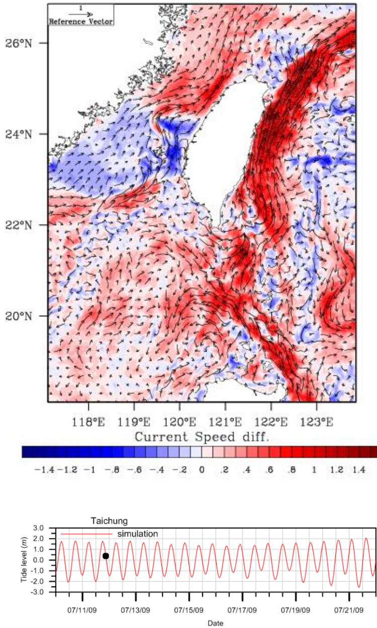
圖 2-25(續) 臺灣海域自綜合洋流與潮流效應之擬真海流流場中扣除潮流效應所得之恆常海流流場(台中港退潮期 2009/07/11 21:00)
