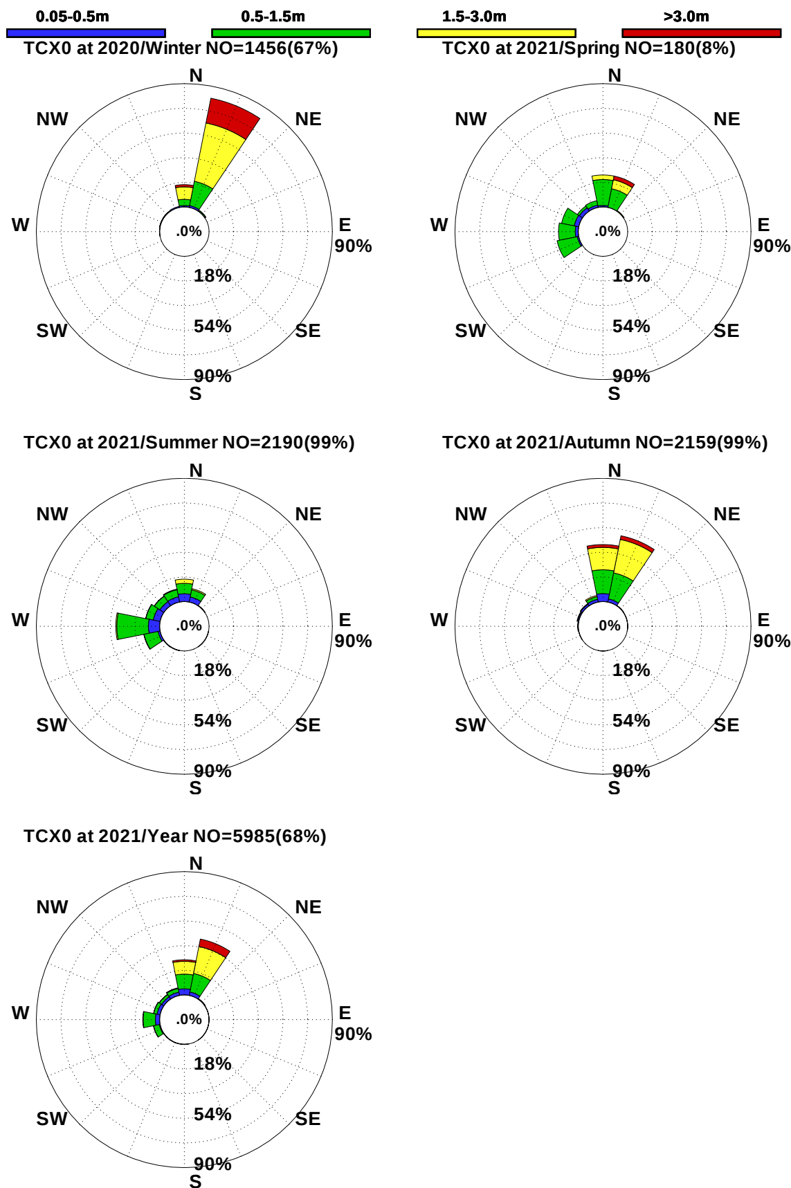
圖9.4b 2021年臺中港每季測站 X 觀測浪玫瑰圖
