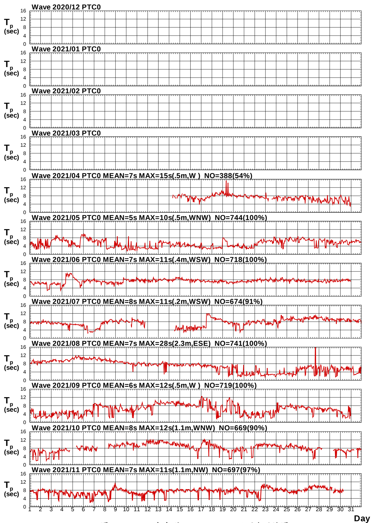
圖8.3b 2021年每月 BDBU01H02站週期歷線圖
