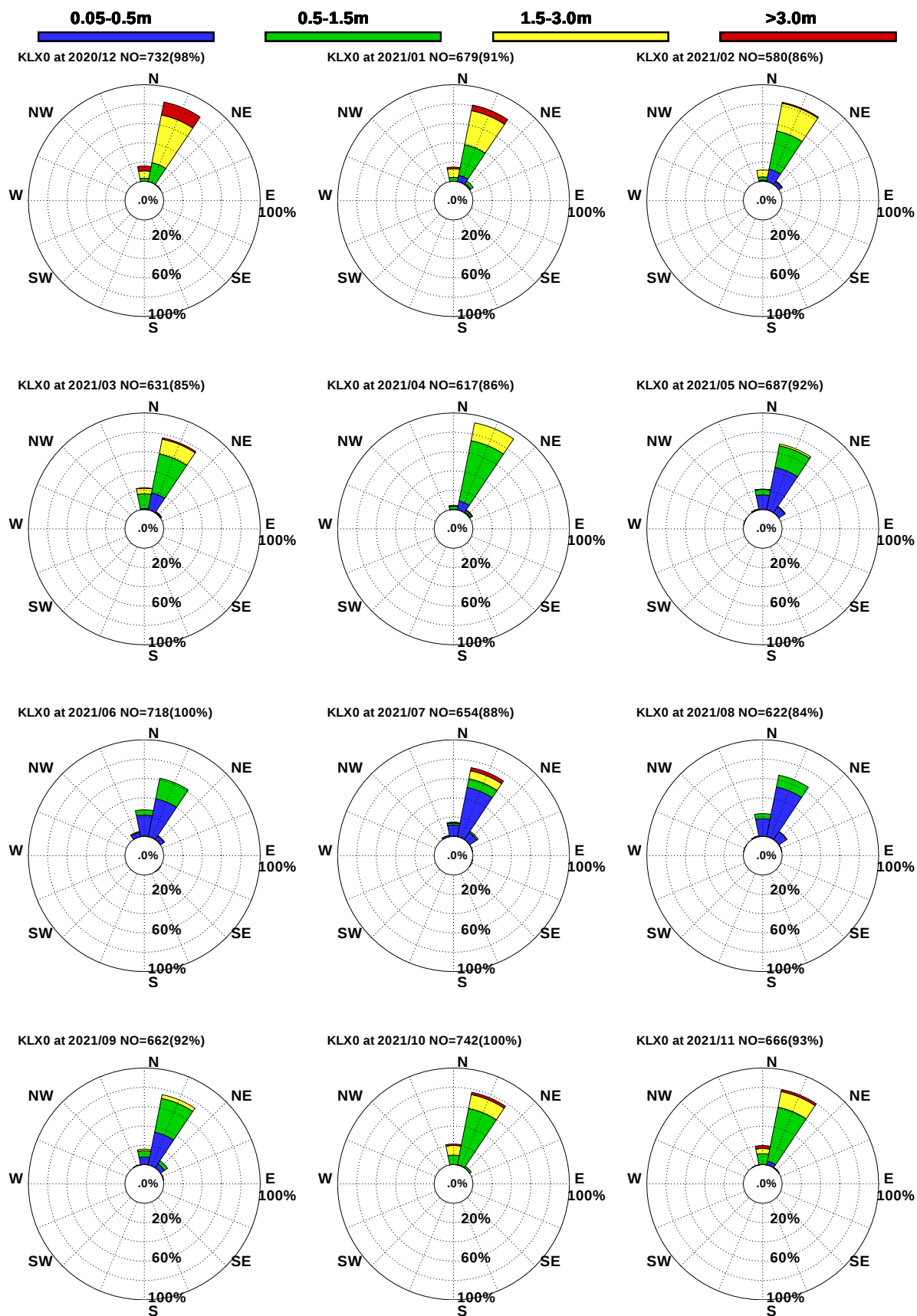
圖3.4a 2021年基隆港每月測站 X 觀測浪玫瑰圖
