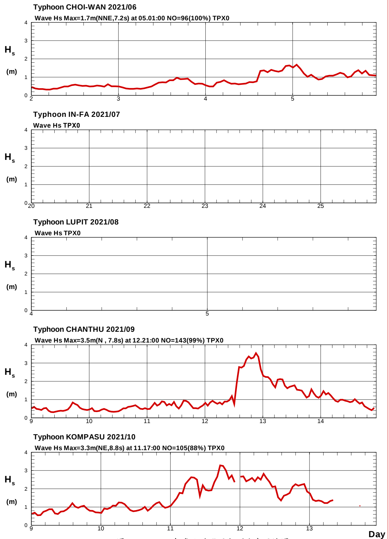
圖2.5a 2021年臺北港颱風觀測波高歷線圖
