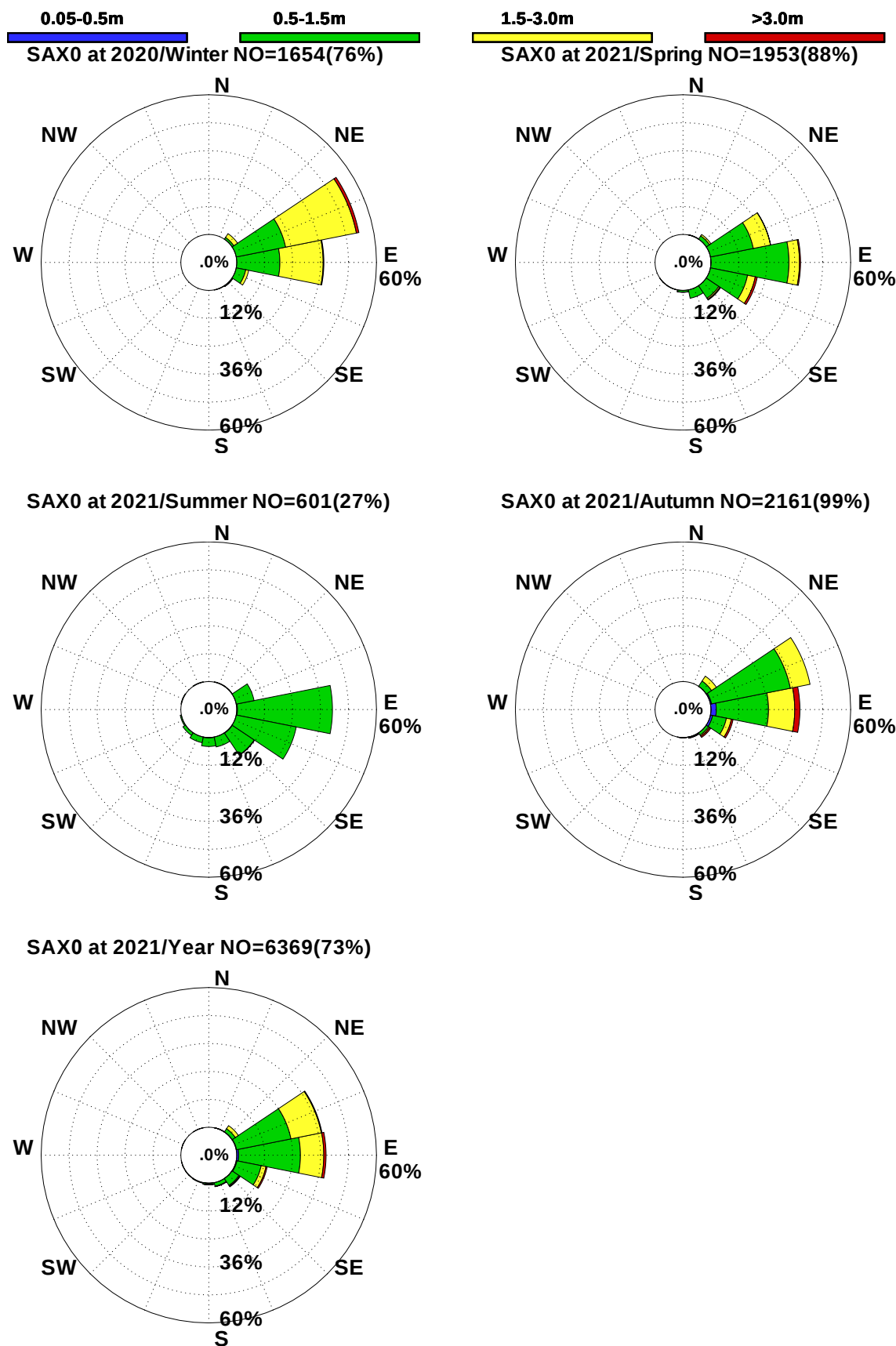
圖4.4b 2021年蘇澳港每季測站 X 觀測浪玫瑰圖
