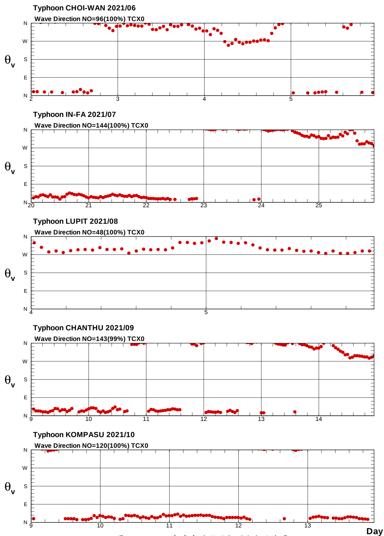
圖9.5b 2021年臺中港颱風觀測波向歷線圖
