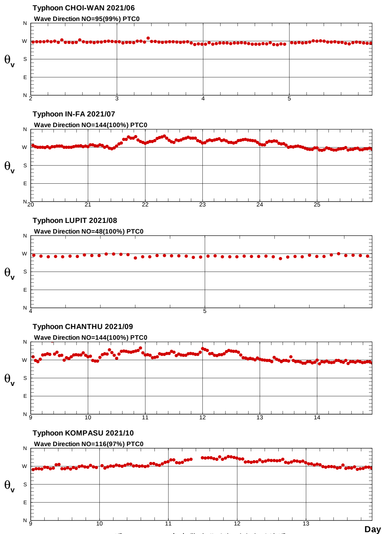
圖8.5b 2021年布袋港颱風觀測波向歷線圖
