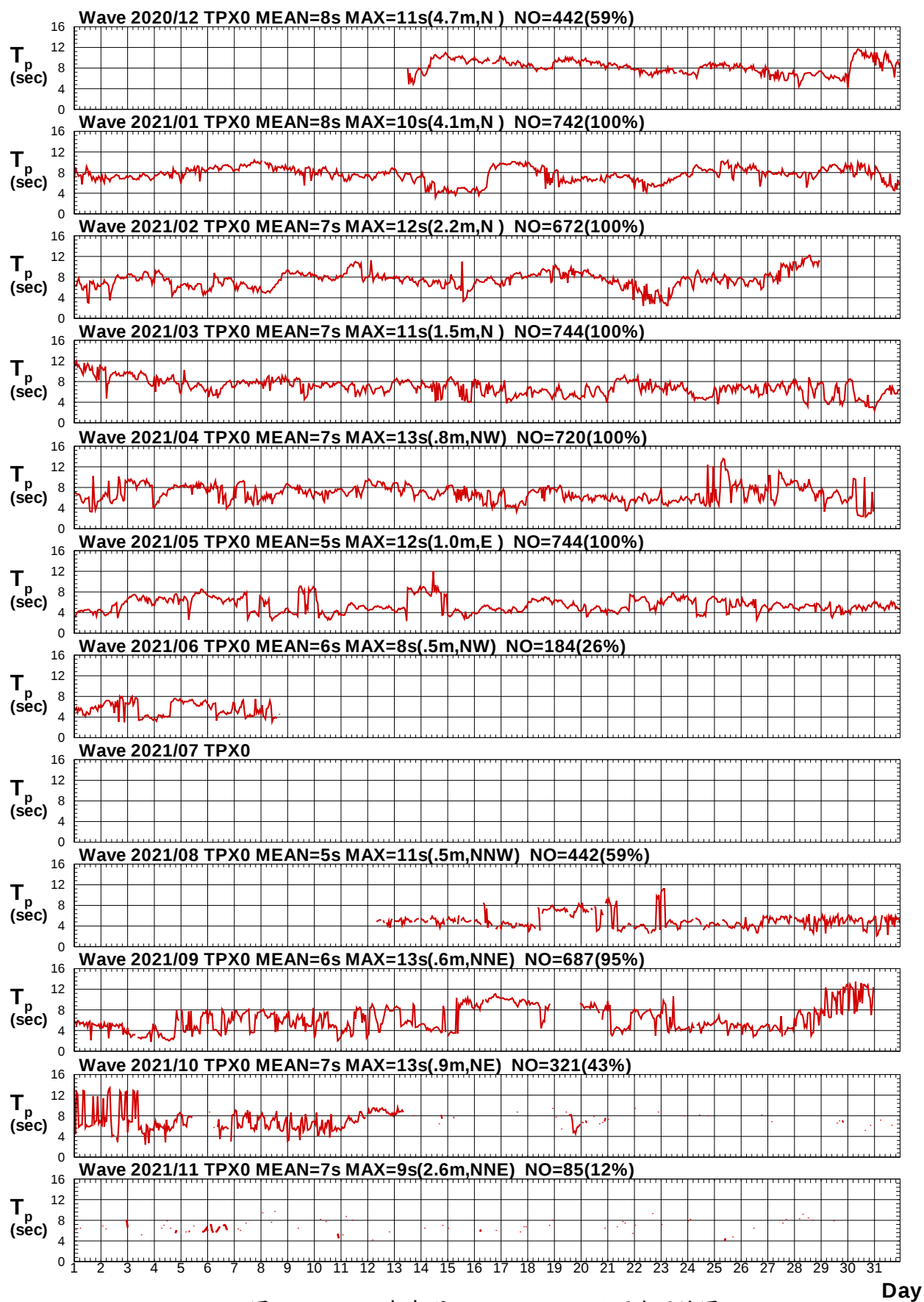
圖2.3b 2021年每月 TPAW01H01 站週期歷線圖
