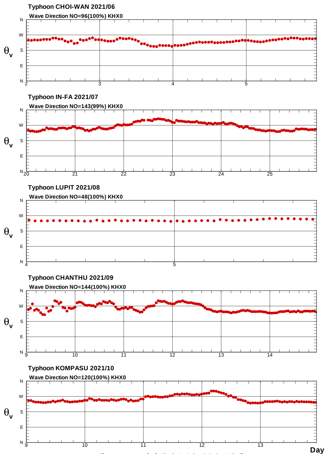
圖6.5b 2021年高雄港颱風觀測波向歷線圖
