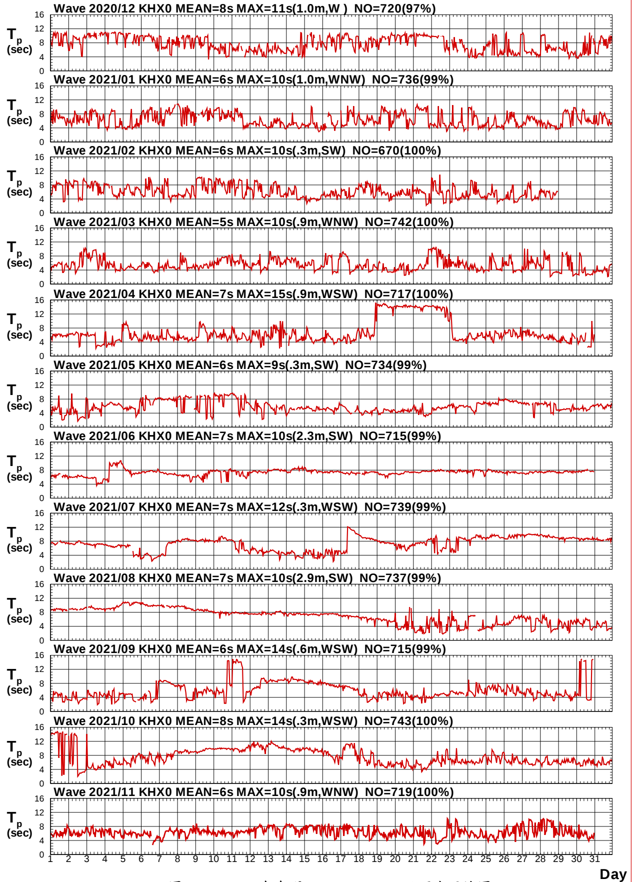
圖6.3b 2021年每月 KHA01H01站週期歷線圖
