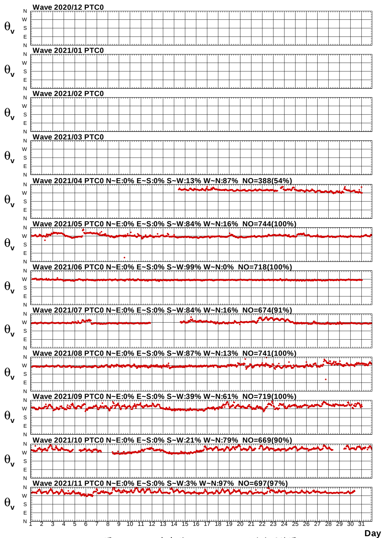
圖8.3c 2021年每月 BDBU01H02站波向歷線圖
