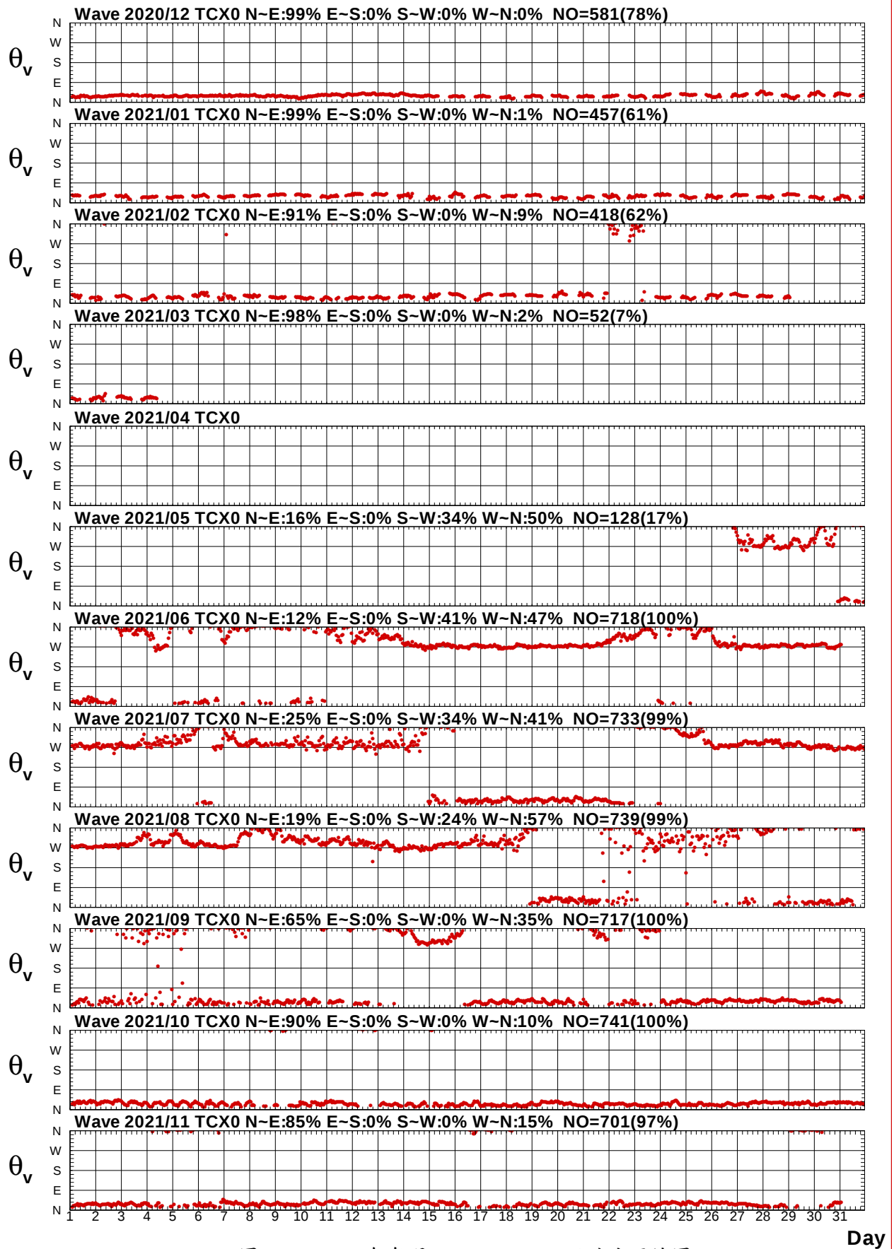
圖9.3c 2021年每月 TCAW01H01站波向歷線圖
