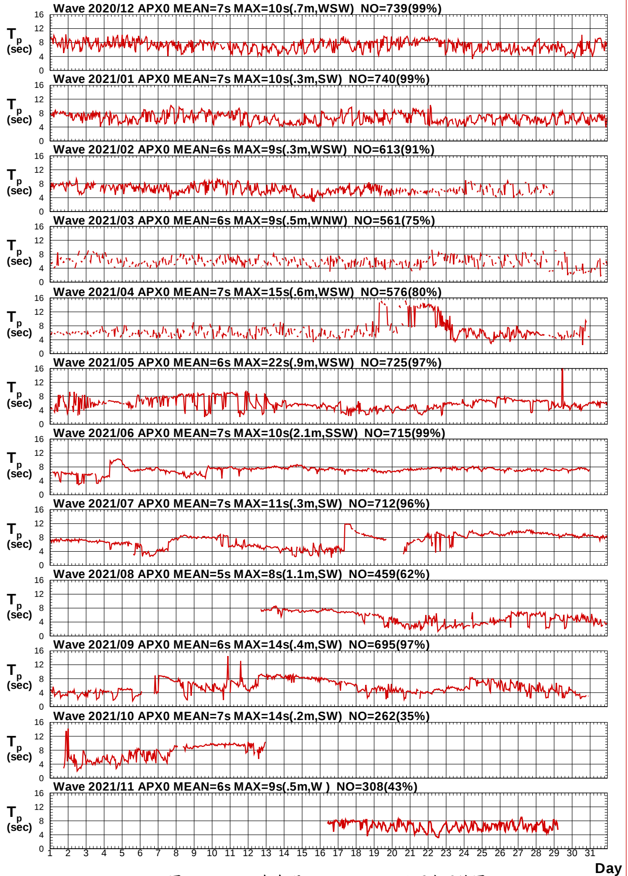
圖7.3b 2021年每月 APAW01H01 站週期歷線圖
