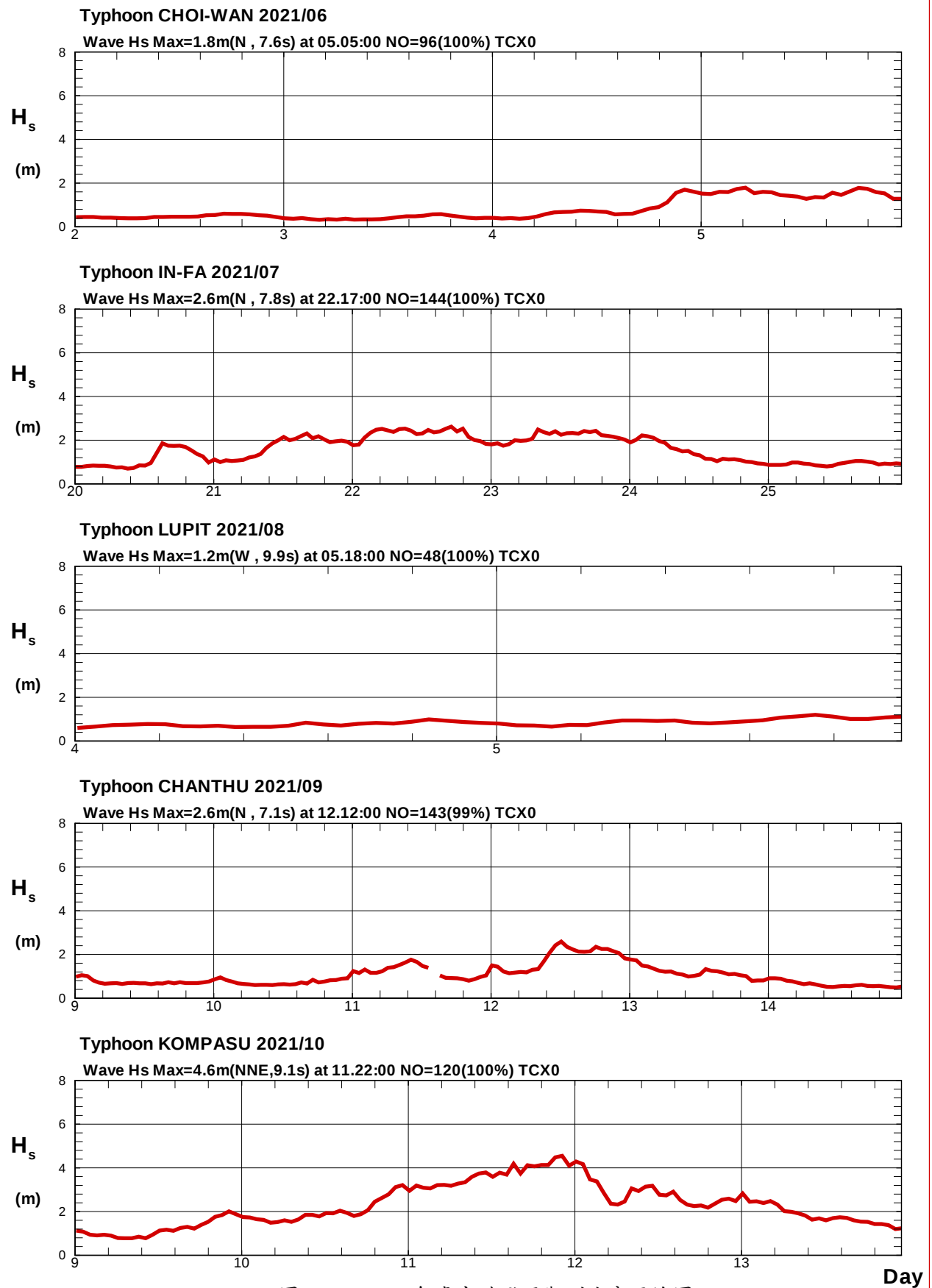
圖9.5a 2021年臺中港颱風觀測波高歷線圖
