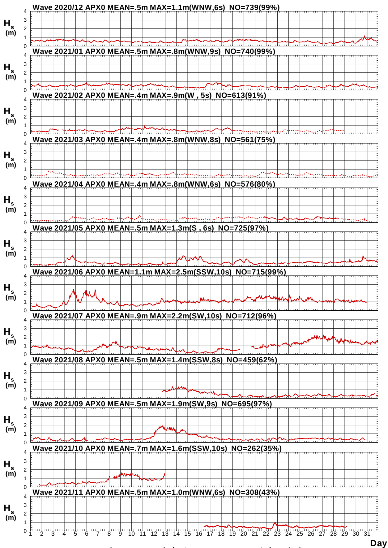
圖7.3a 2021年每月 APAW01H01站波高歷線圖
