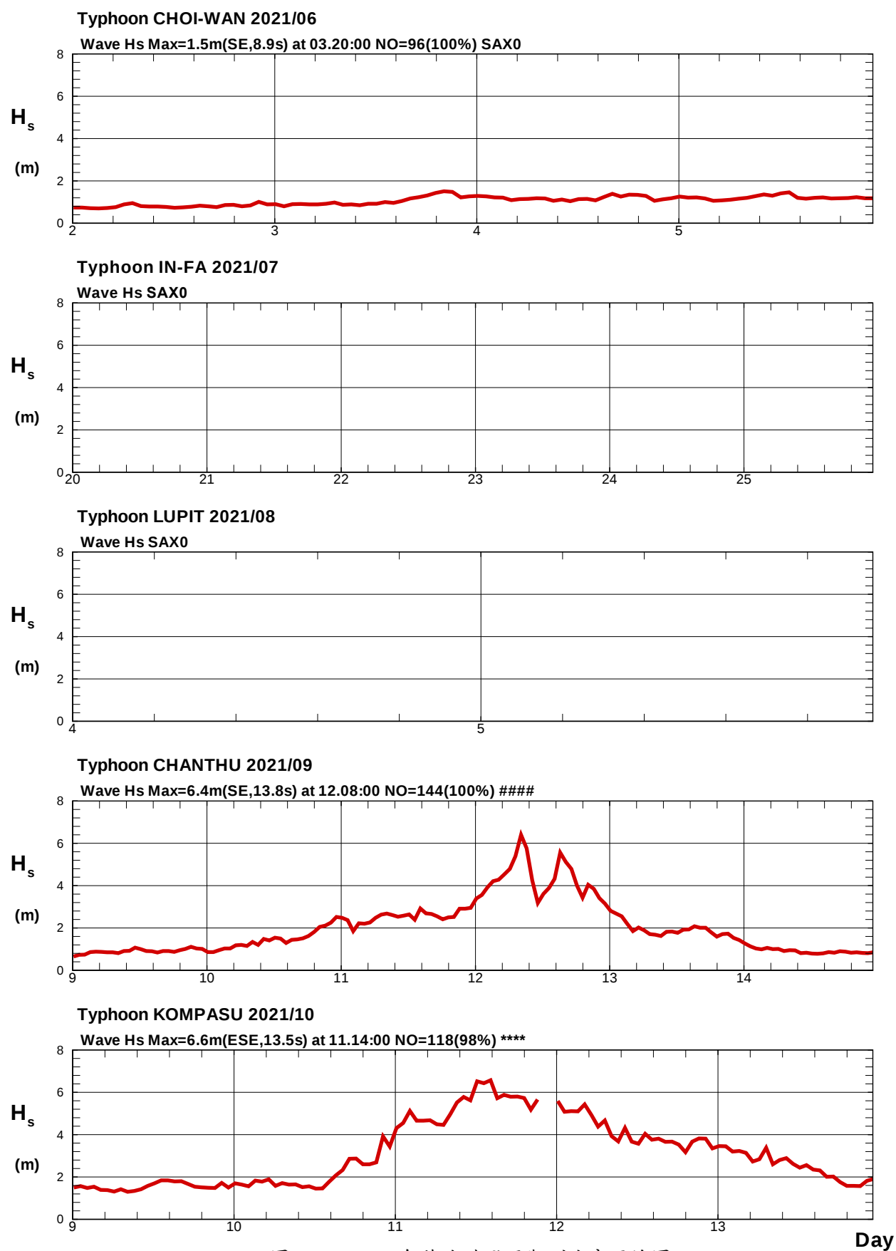
圖4.5a 2021年蘇澳港颱風觀測波高歷線圖
