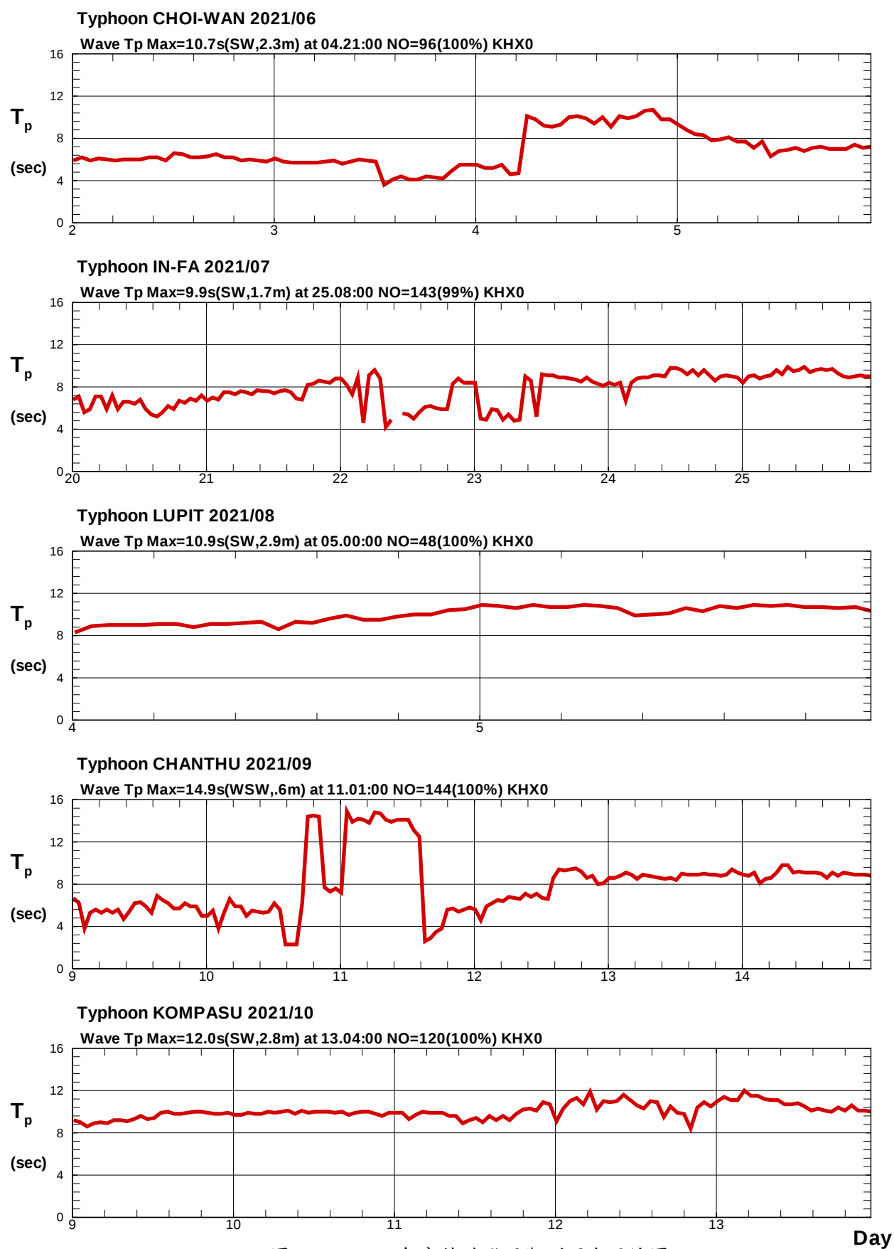
圖6.5c 2021年高雄港颱風觀測週期歷線圖
