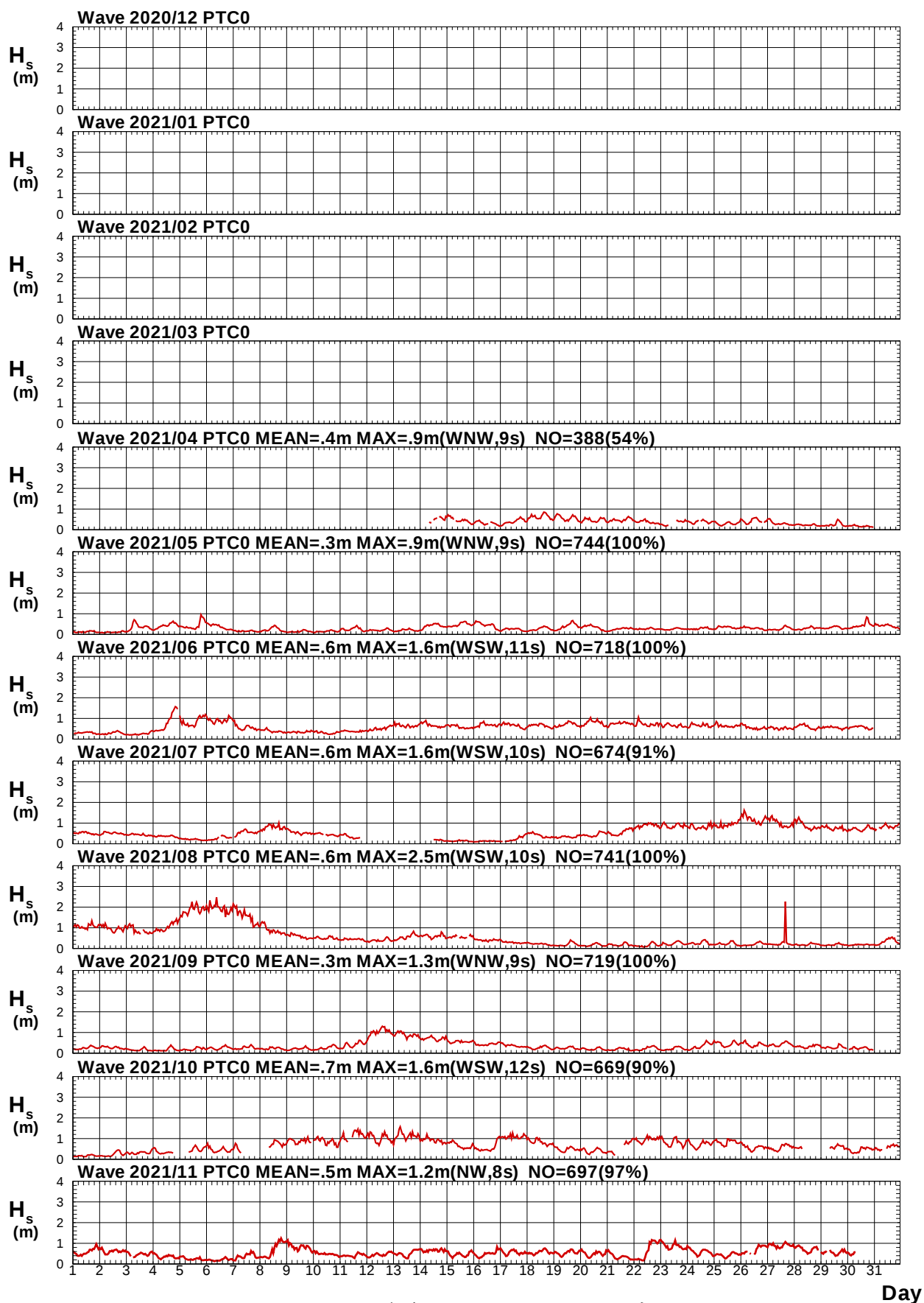
圖8.3a 2021年每月 BDBU01H02站波高歷線圖
