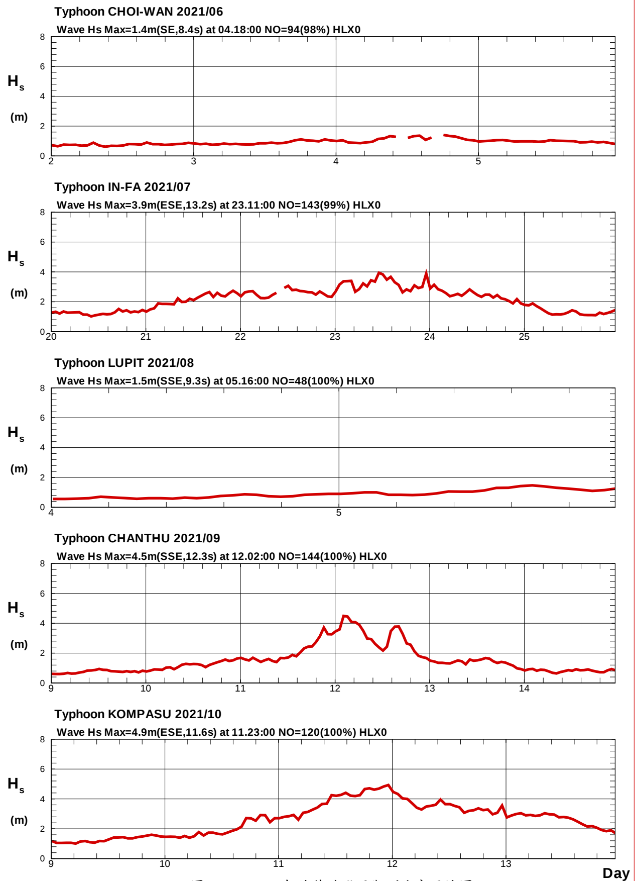
圖5.5a 2021年花蓮港颱風觀測波高歷線圖
