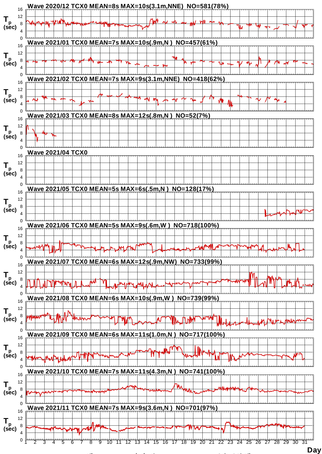
圖9.3b 2021年每月 TCAW01H01站週期歷線圖
