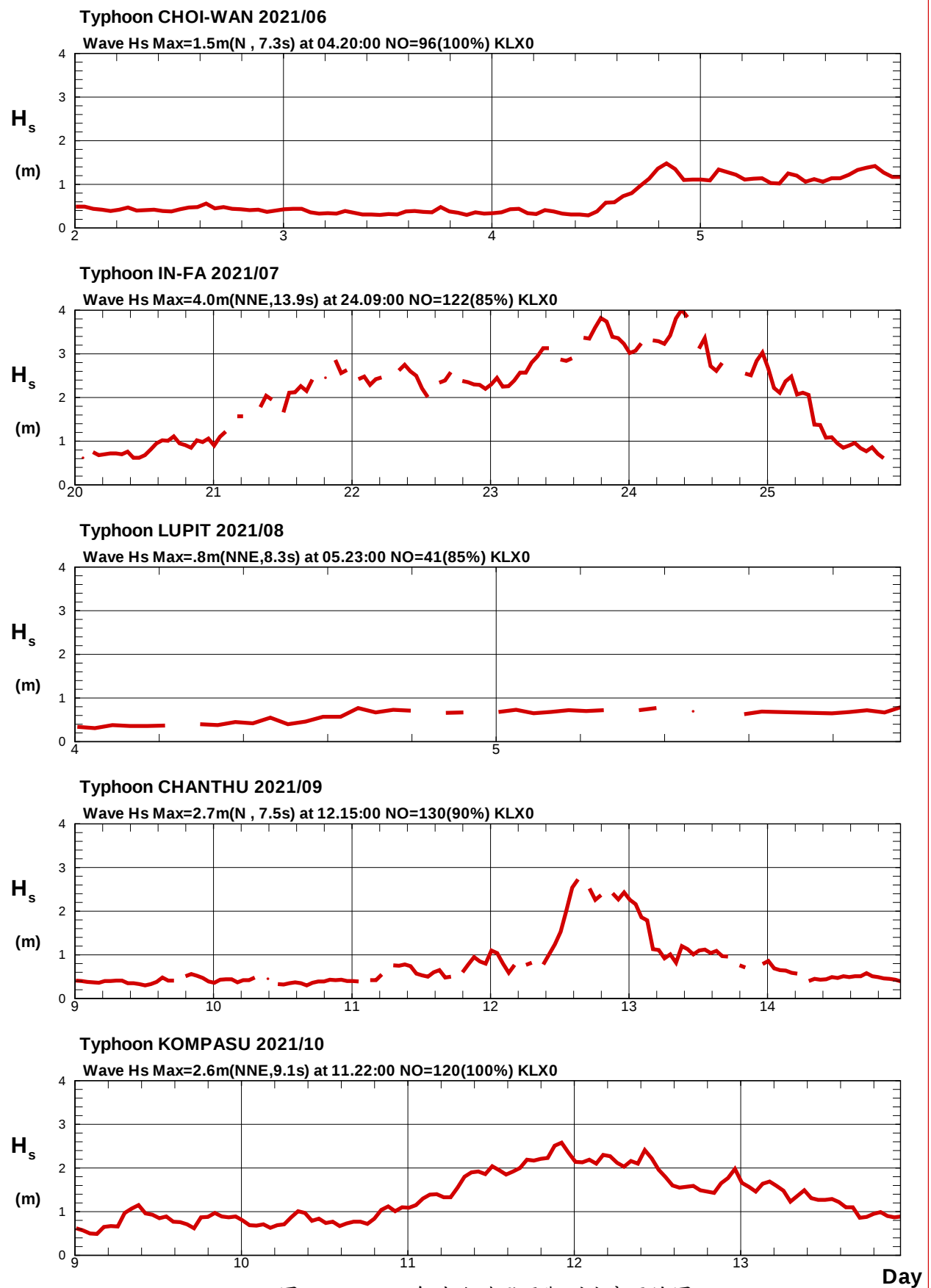
圖3.5a 2021年基隆港颱風觀測波高歷線圖
