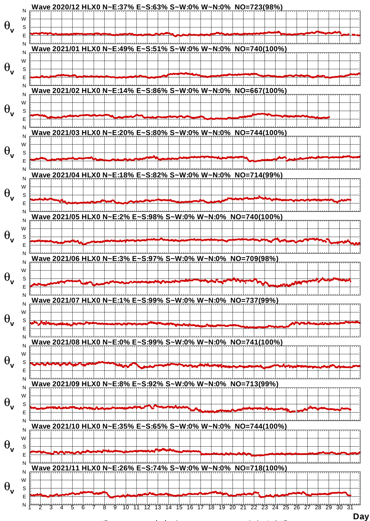
圖5.3c 2021年每月 HLAW01H01站波向歷線圖
