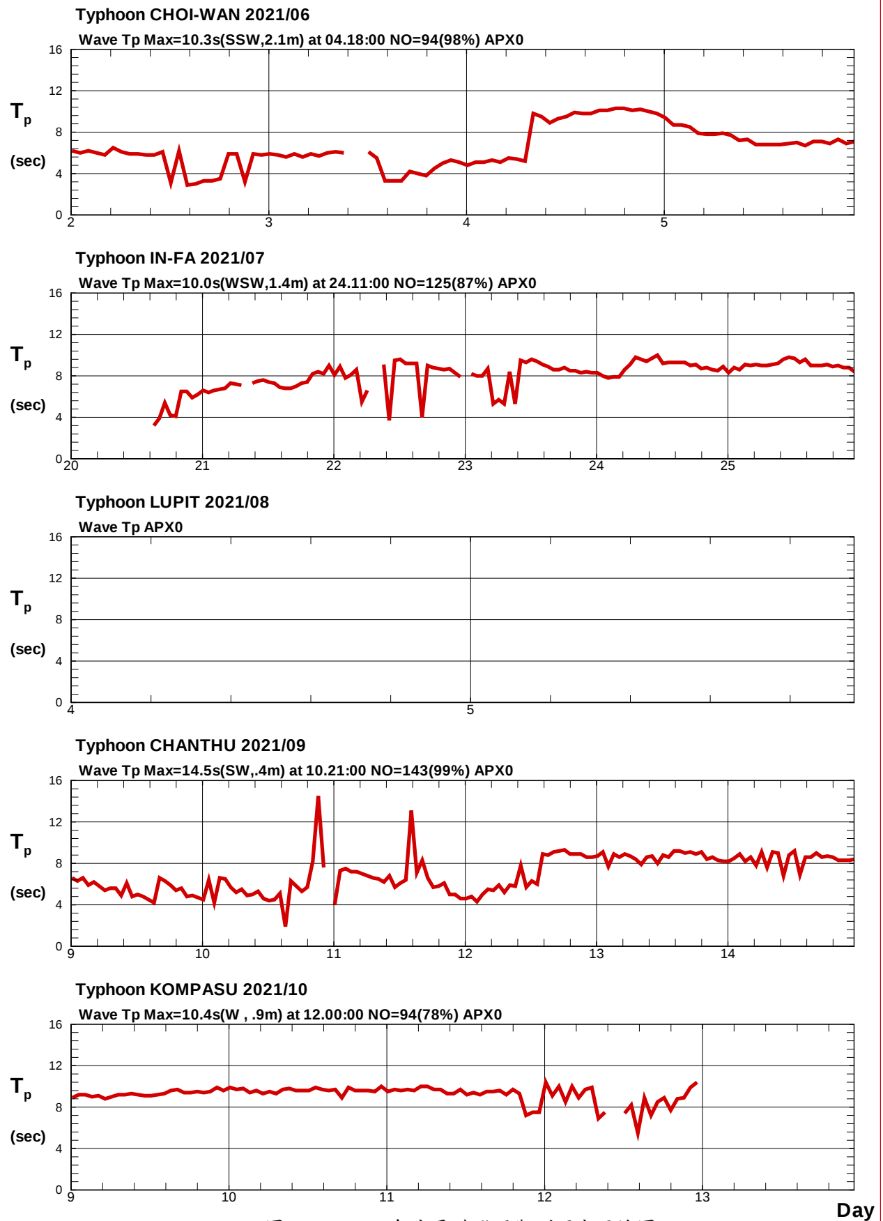
圖7.5c 2021年安平港颱風觀測週期歷線圖
