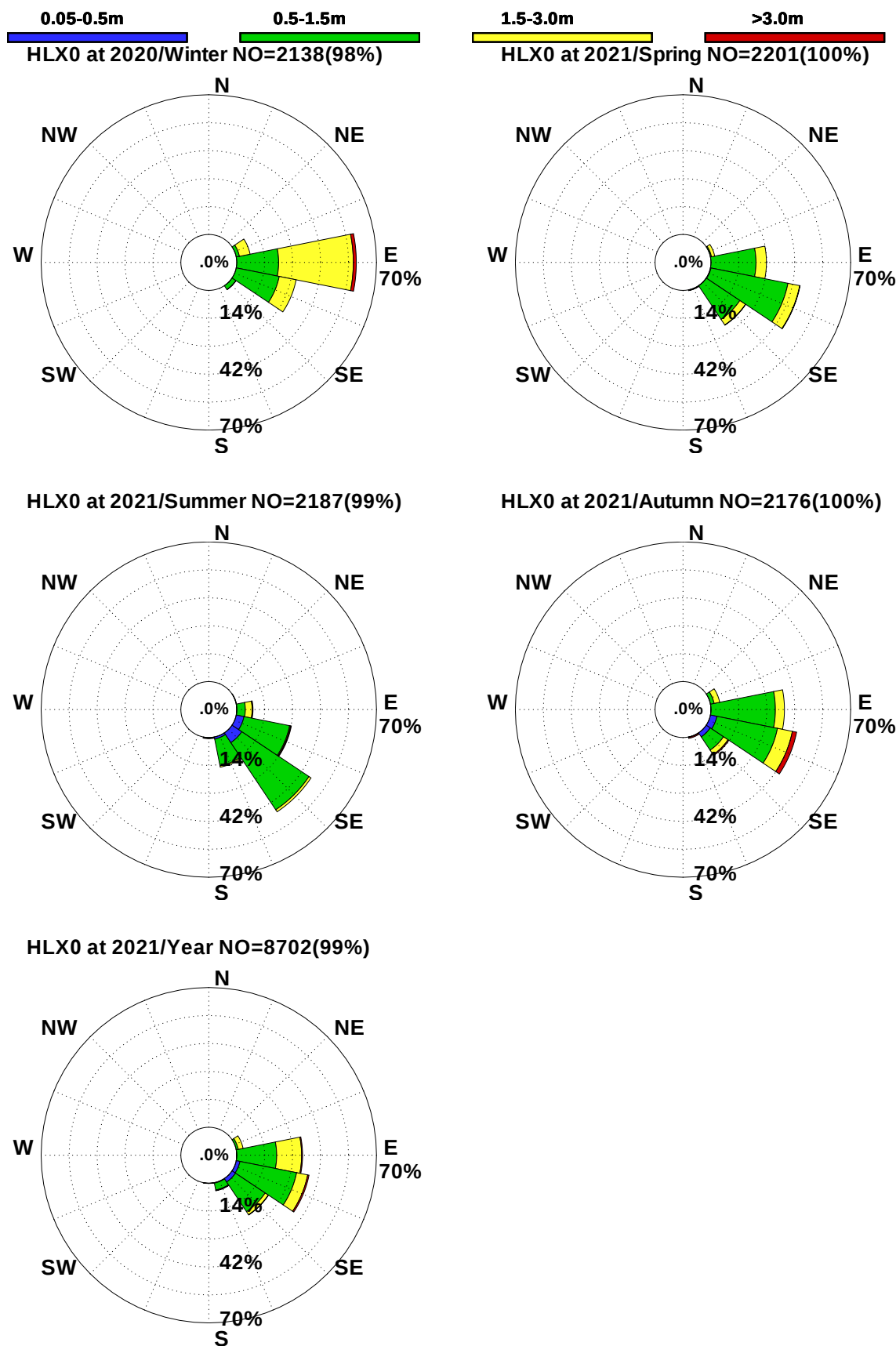
圖5.4b 2021年花蓮港每季測站 X 觀測浪玫瑰圖
