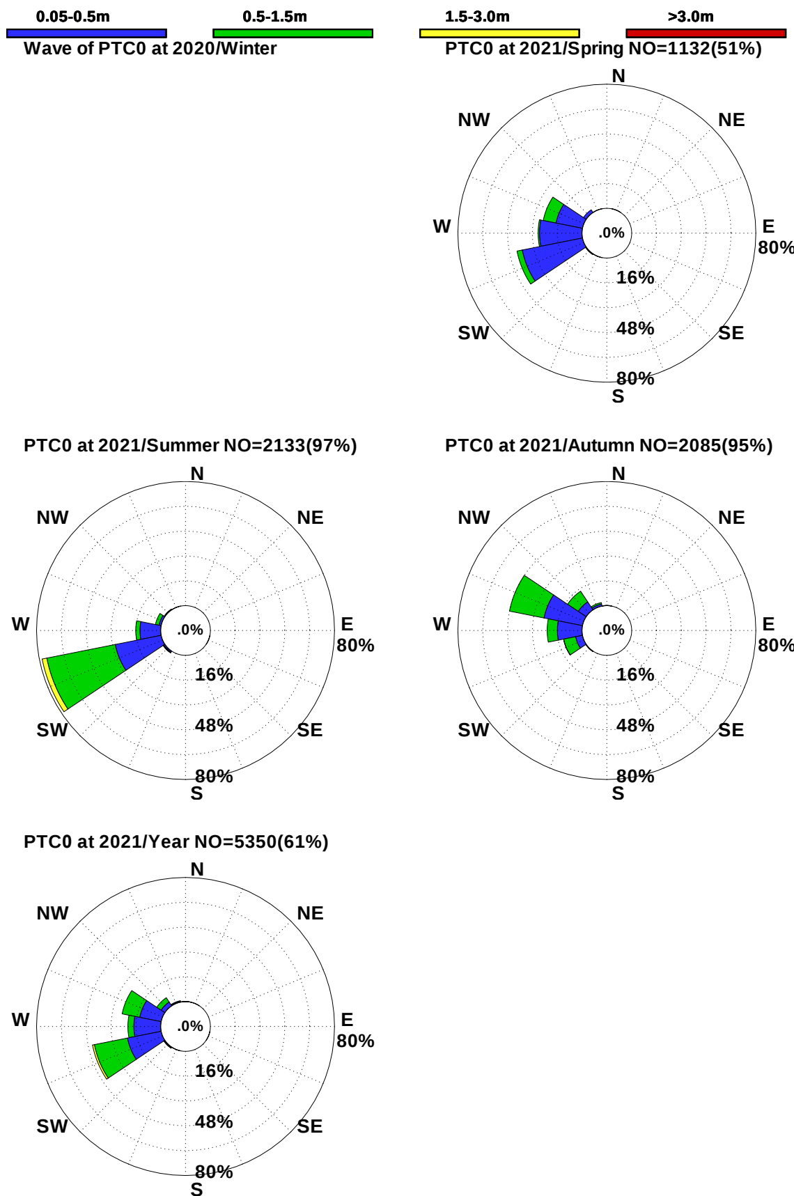
圖8.4b 2021年布袋港每季測站 C 觀測浪玫瑰圖
