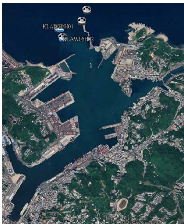
圖 3.1 基隆港波浪測站位置圖
