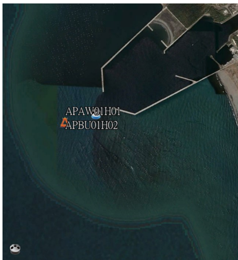
圖 7.1 安平港波浪測站位置圖
