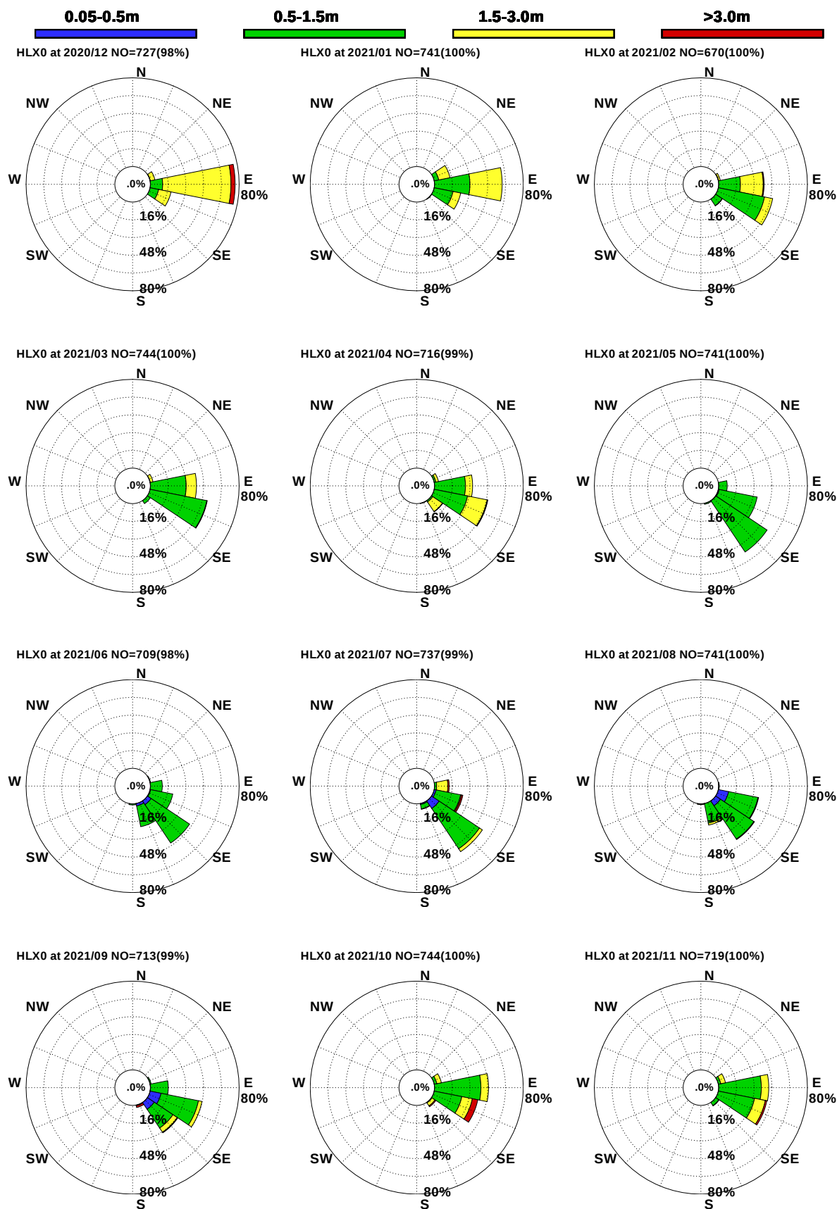
圖5.4a 2021年花蓮港每月測站 X 觀測浪玫瑰圖
