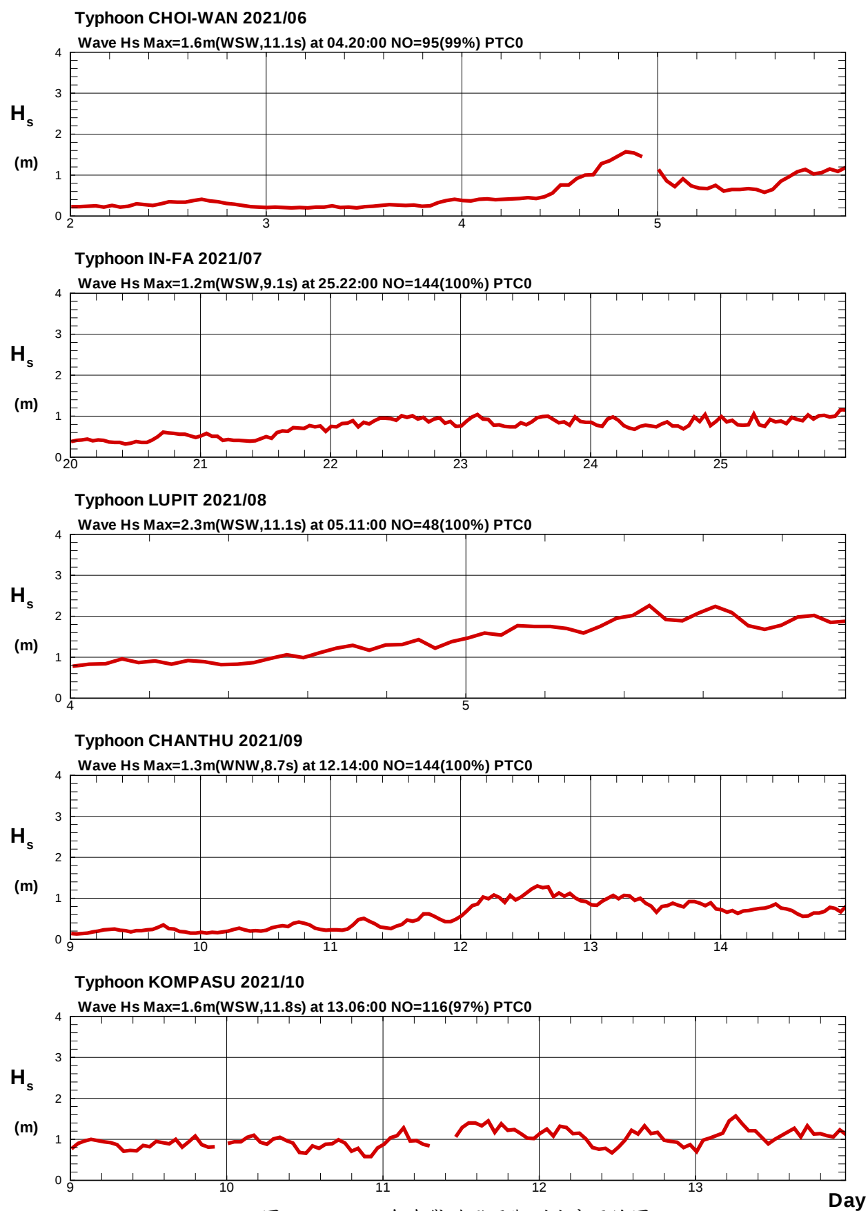
圖8.5a 2021年布袋港颱風觀測波高歷線圖
