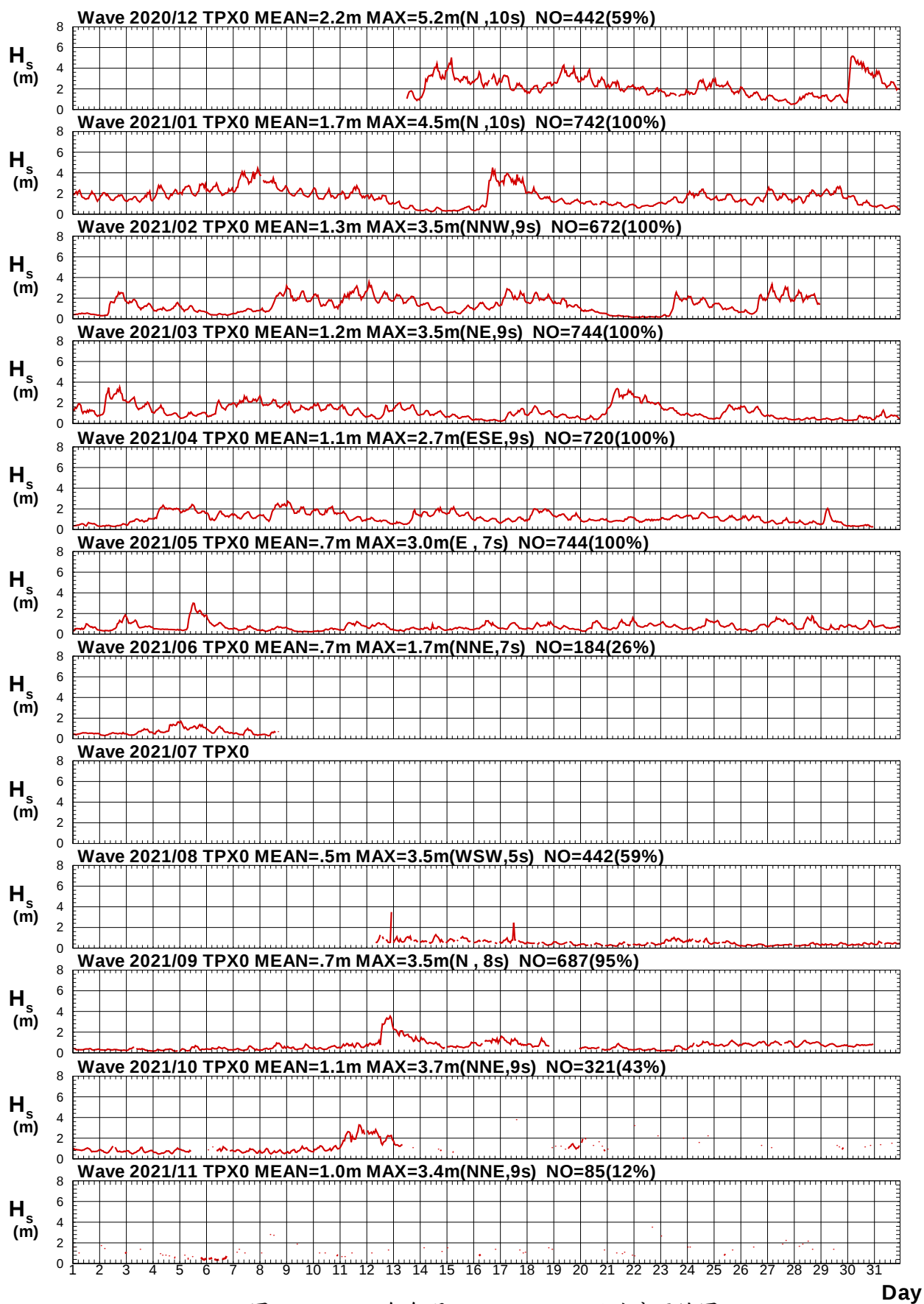
圖2.3a 2021年每月 TPAW01H01站波高歷線圖
