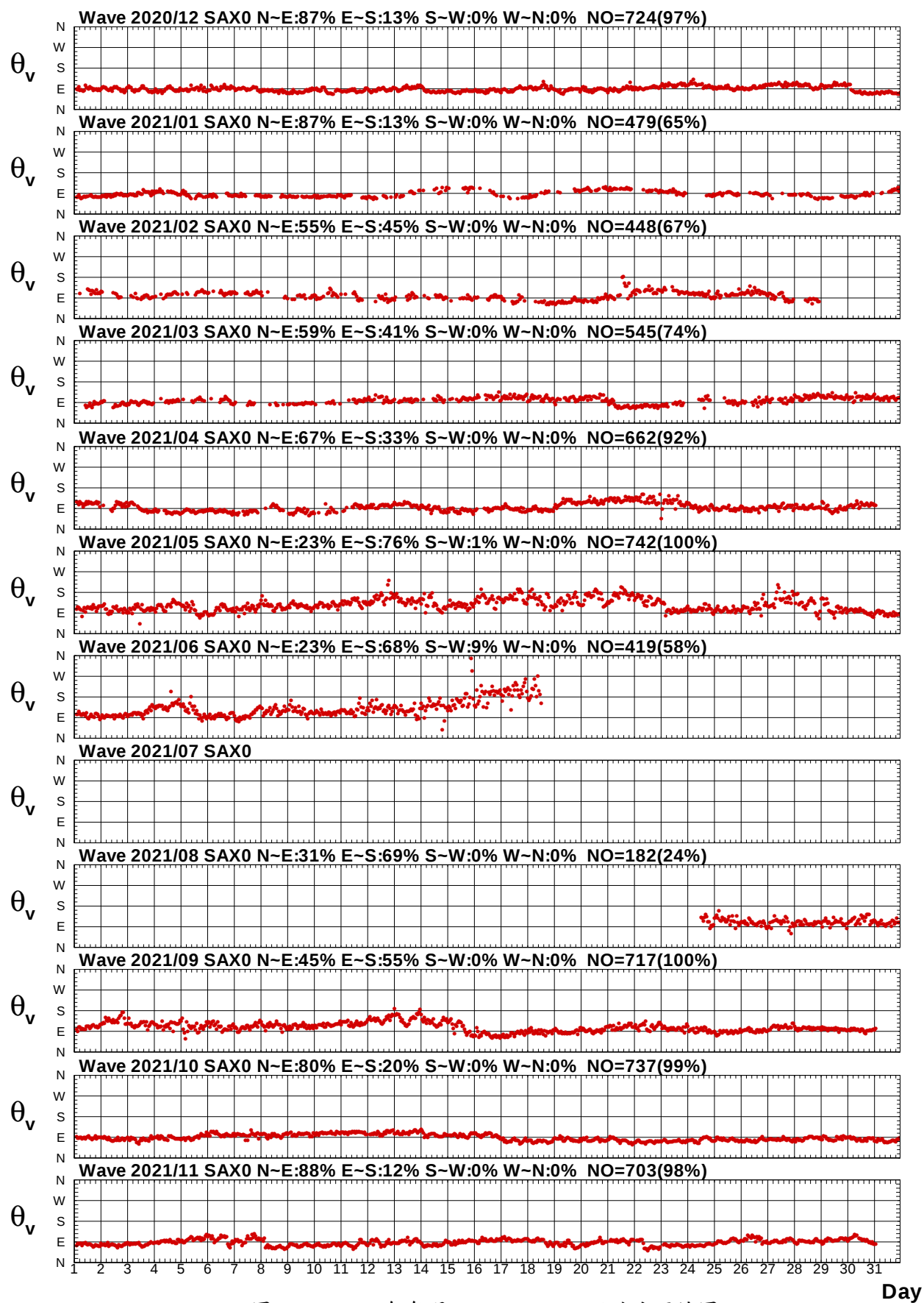
圖4.3c 2021年每月 SAAW01H01站波向歷線圖
