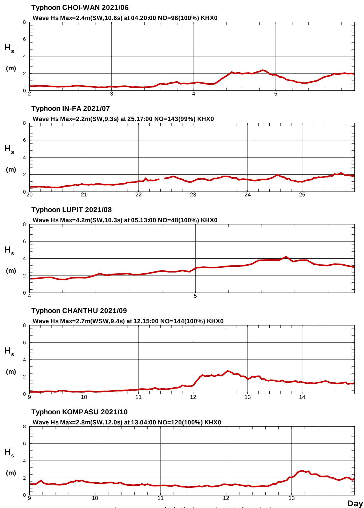
圖6.5a 2021年高雄港颱風觀測波高歷線圖
