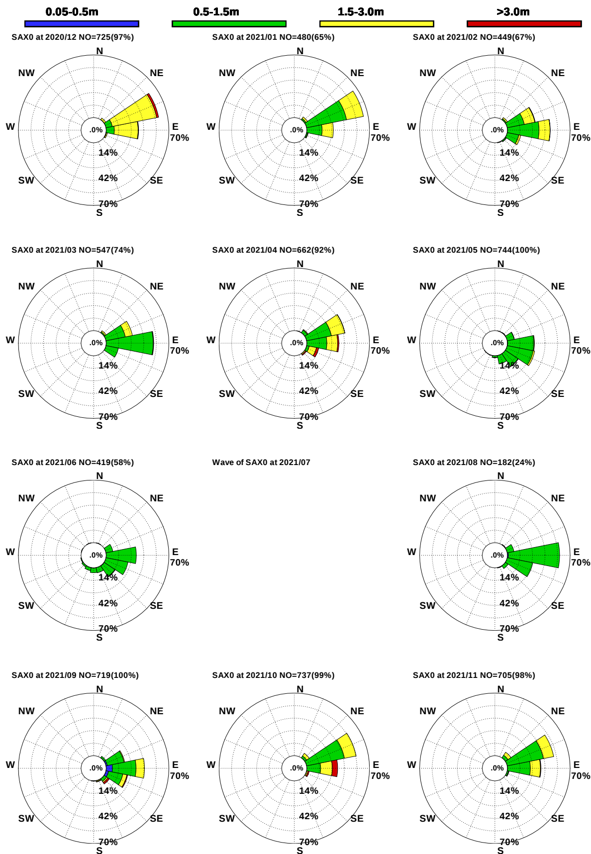
圖4.4a 2021年蘇澳港每月測站 X 觀測浪玫瑰圖
