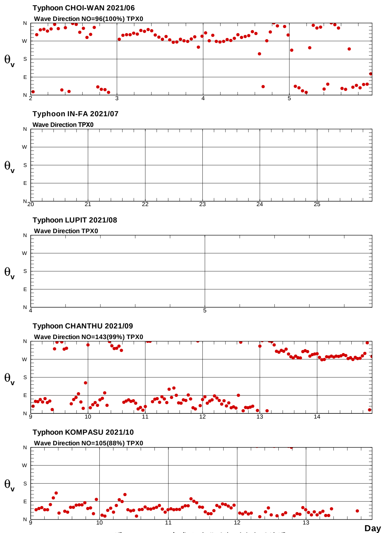
圖2.5b 2021年臺北港颱風觀測波向歷線圖
