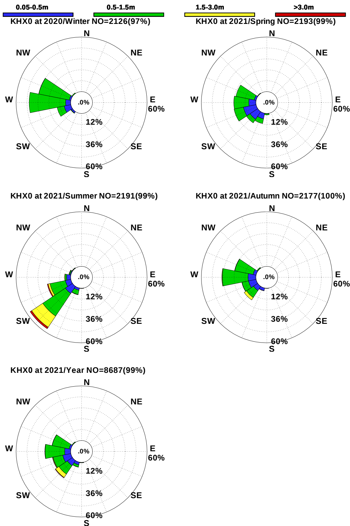
圖6.4b 2021年高雄港每季測站 X 觀測浪玫瑰圖
