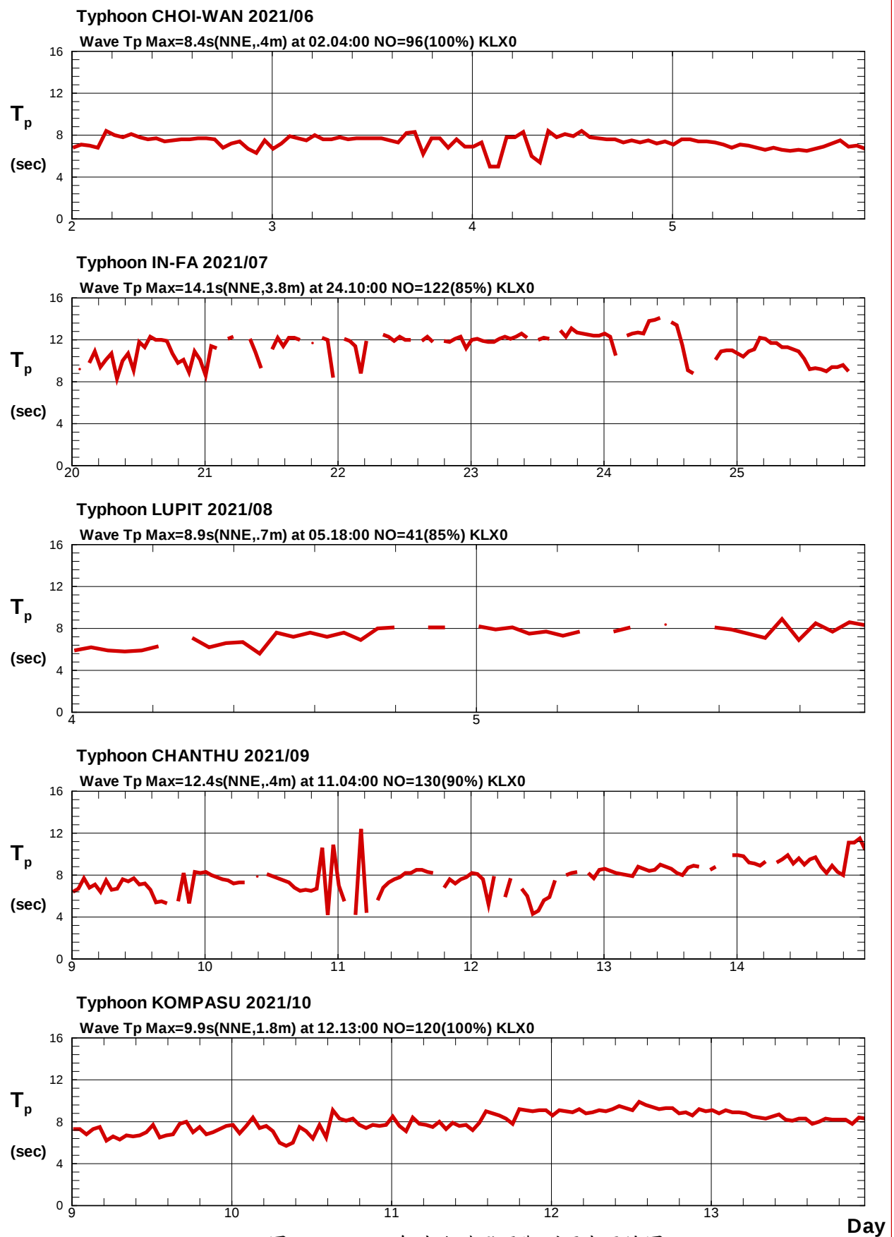
圖3.5c 2021年基隆港颱風觀測週期歷線圖
