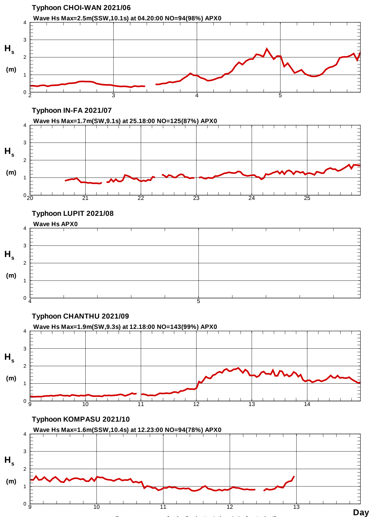
圖7.5a 2021年安平港颱風觀測波高歷線圖
