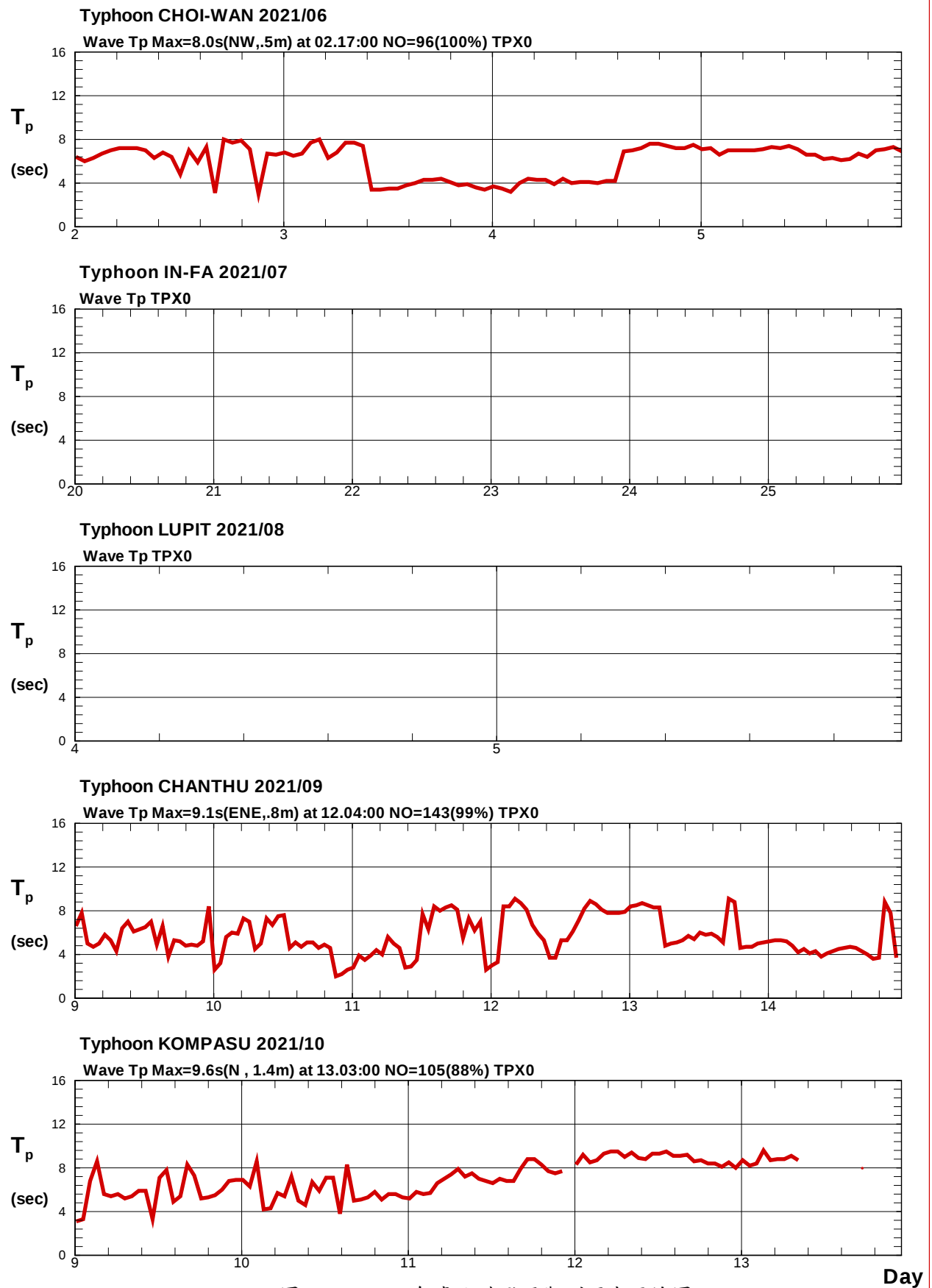
圖2.5c 2021年臺北港颱風觀測週期歷線圖
