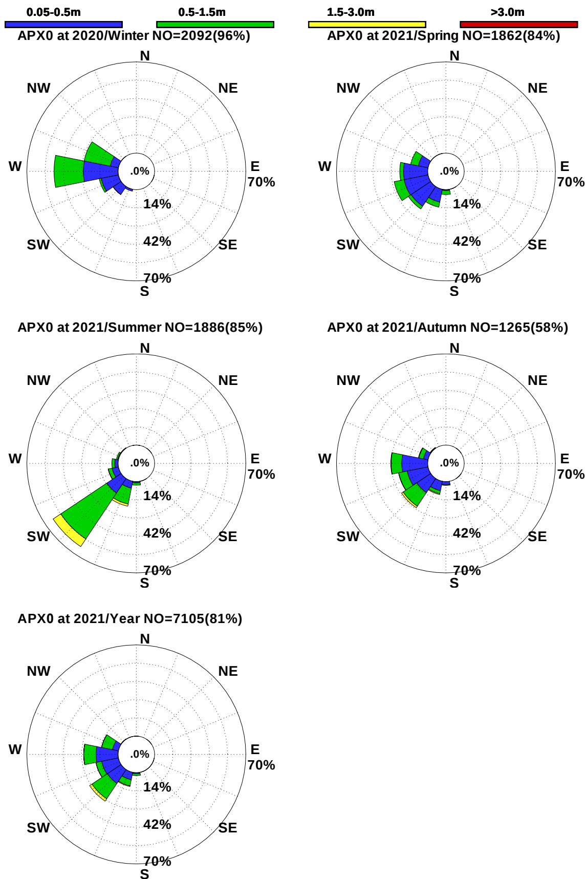
圖7.4b 2021年安平港每季測站 X 觀測浪玫瑰圖
