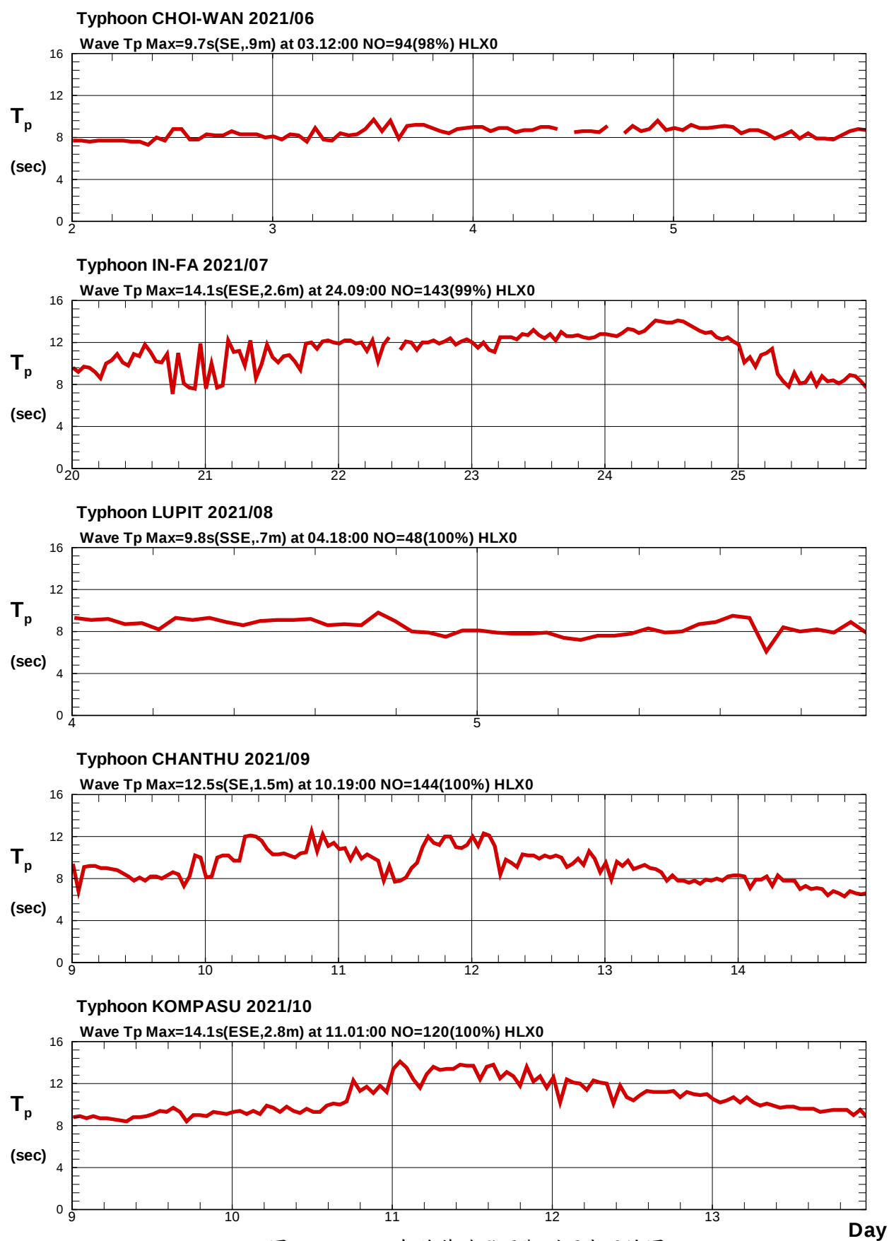
圖5.5c 2021年花蓮港颱風觀測週期歷線圖
