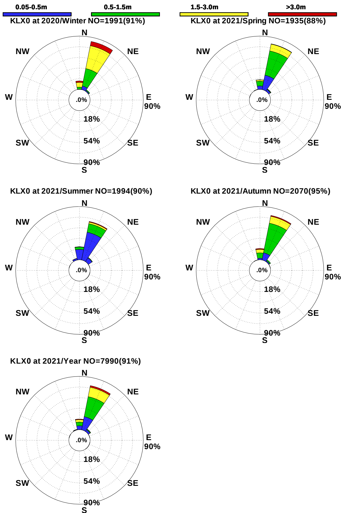
圖3.4b 2021年基隆港每季測站 X 觀測浪玫瑰圖
