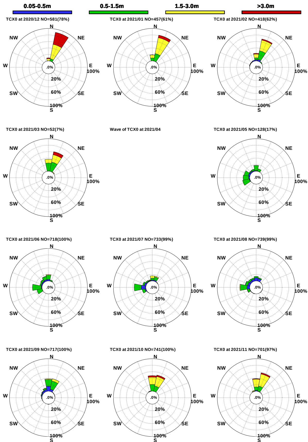
圖9.4a 2021年臺中港每月測站 X 觀測浪玫瑰圖
