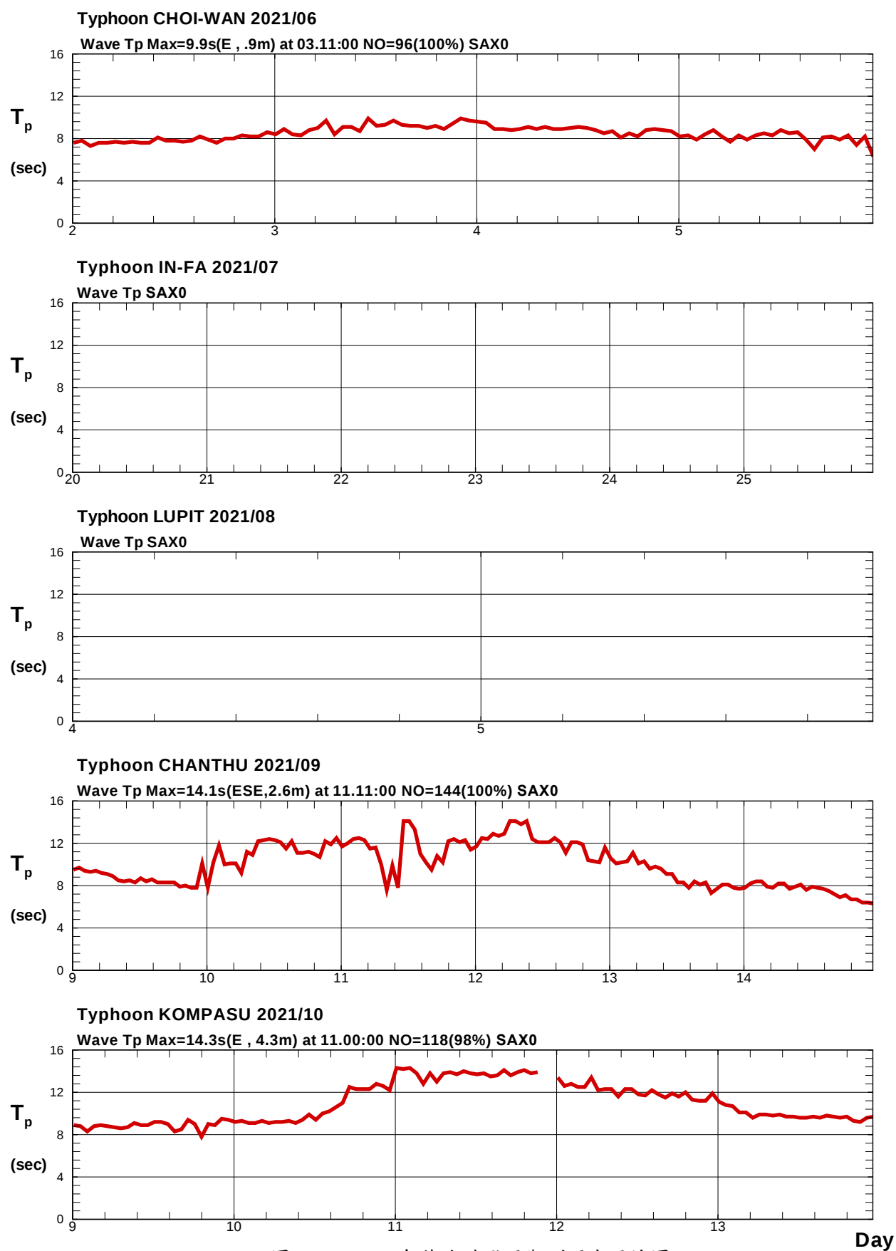
圖4.5c 2021年蘇澳港颱風觀測週期歷線圖
