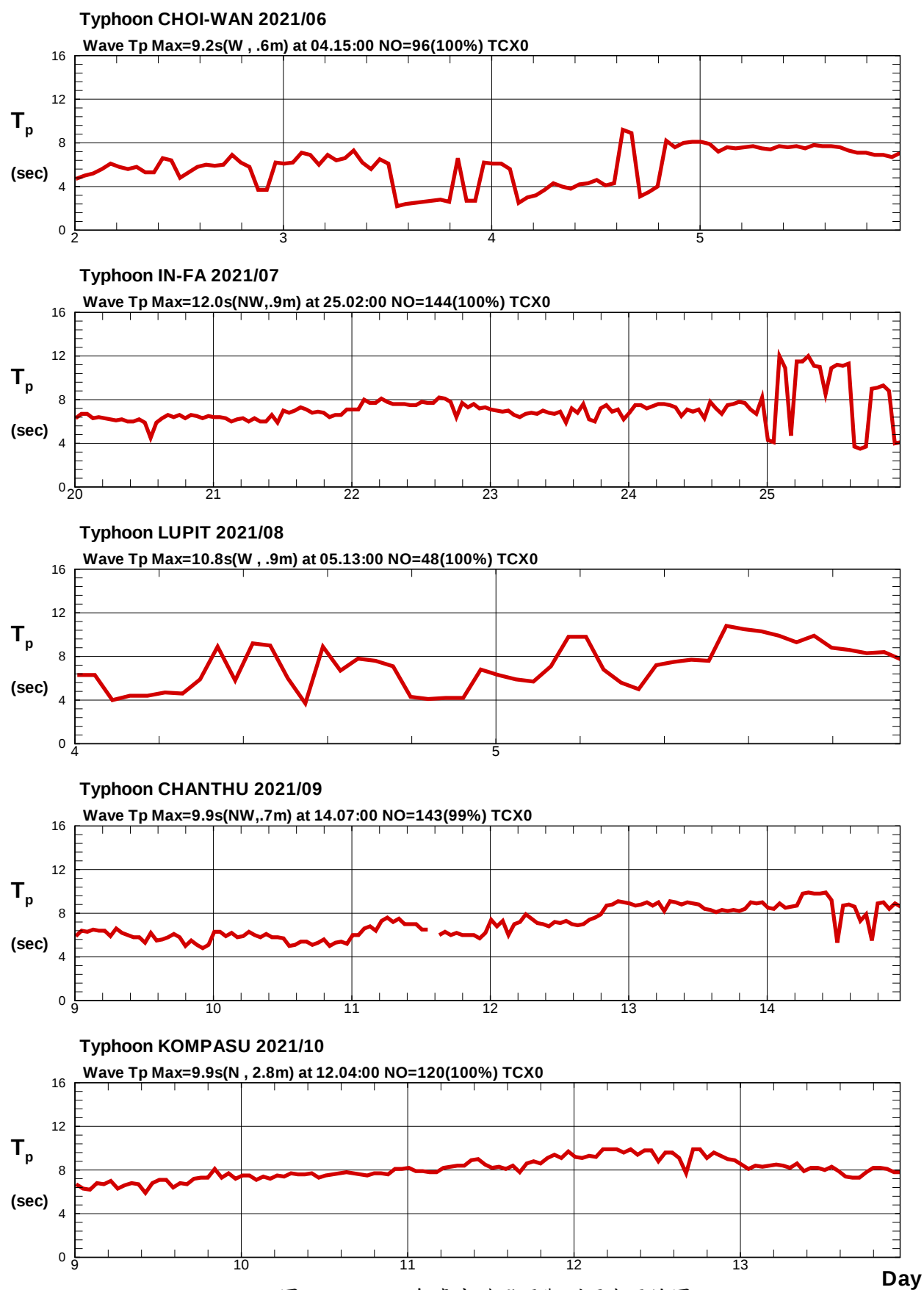
圖9.5c 2021年臺中港颱風觀測週期歷線圖
