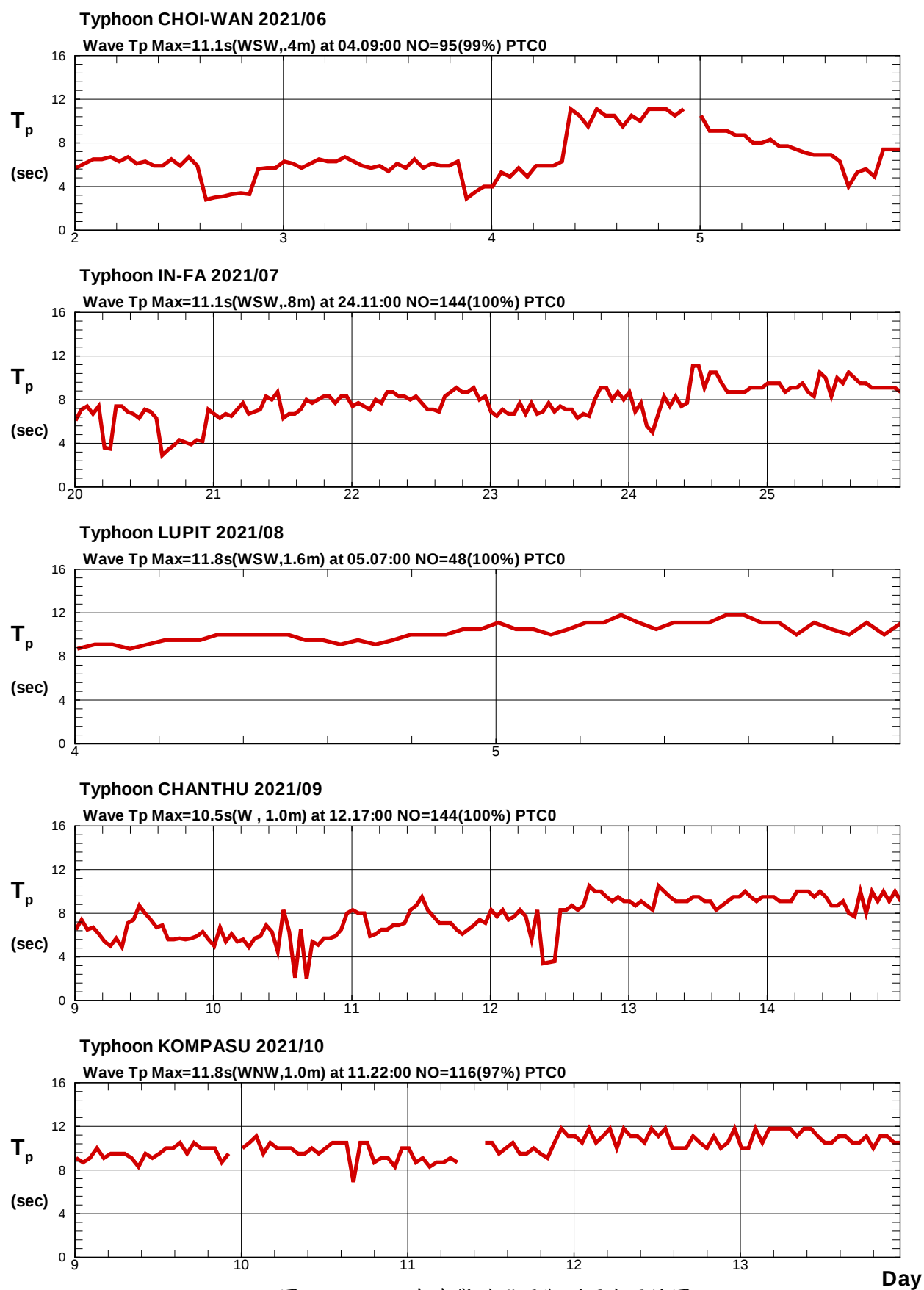
圖8.5c 2021年布袋港颱風觀測週期歷線圖
