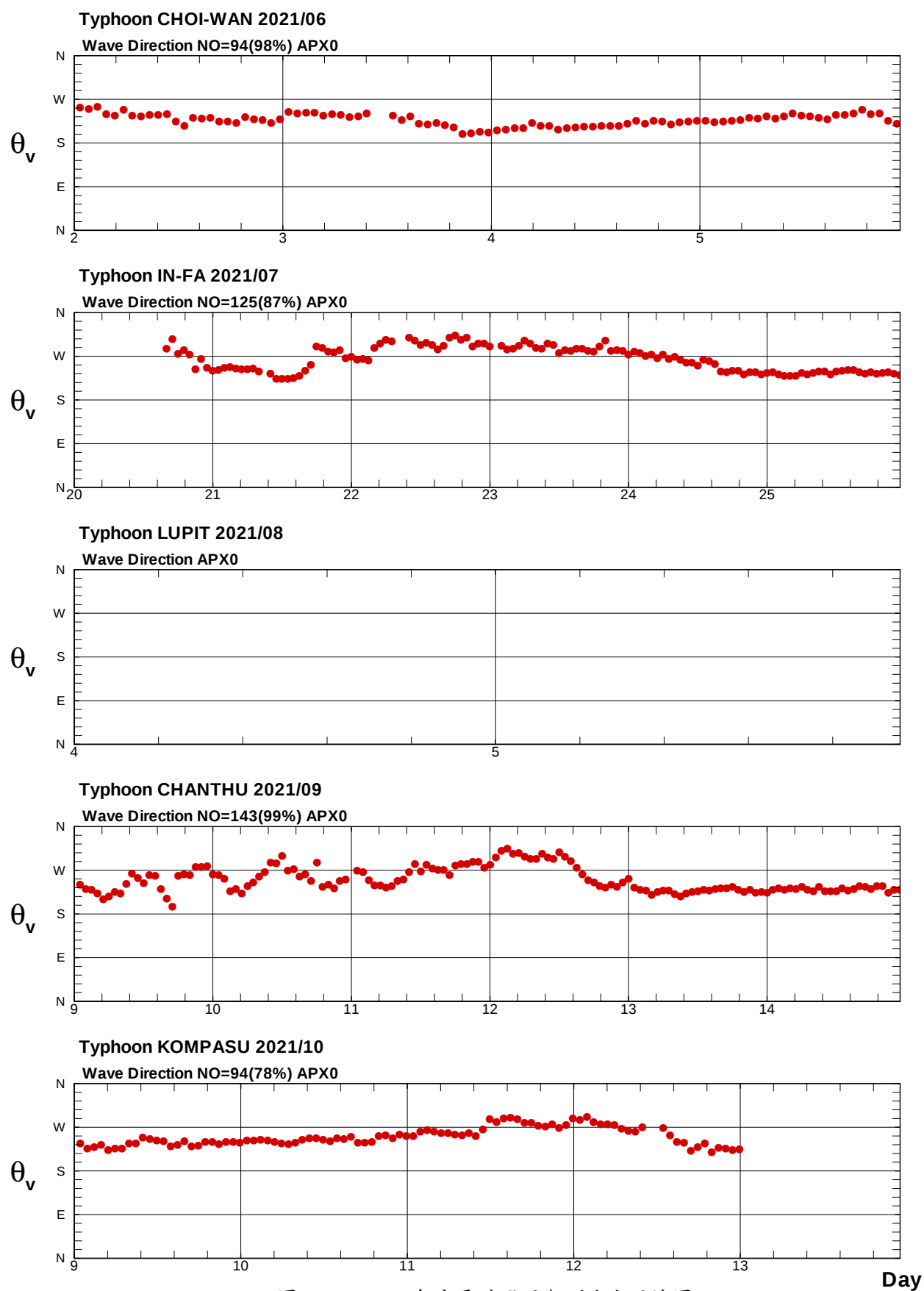
圖7.5b 2021年安平港颱風觀測波向歷線圖
