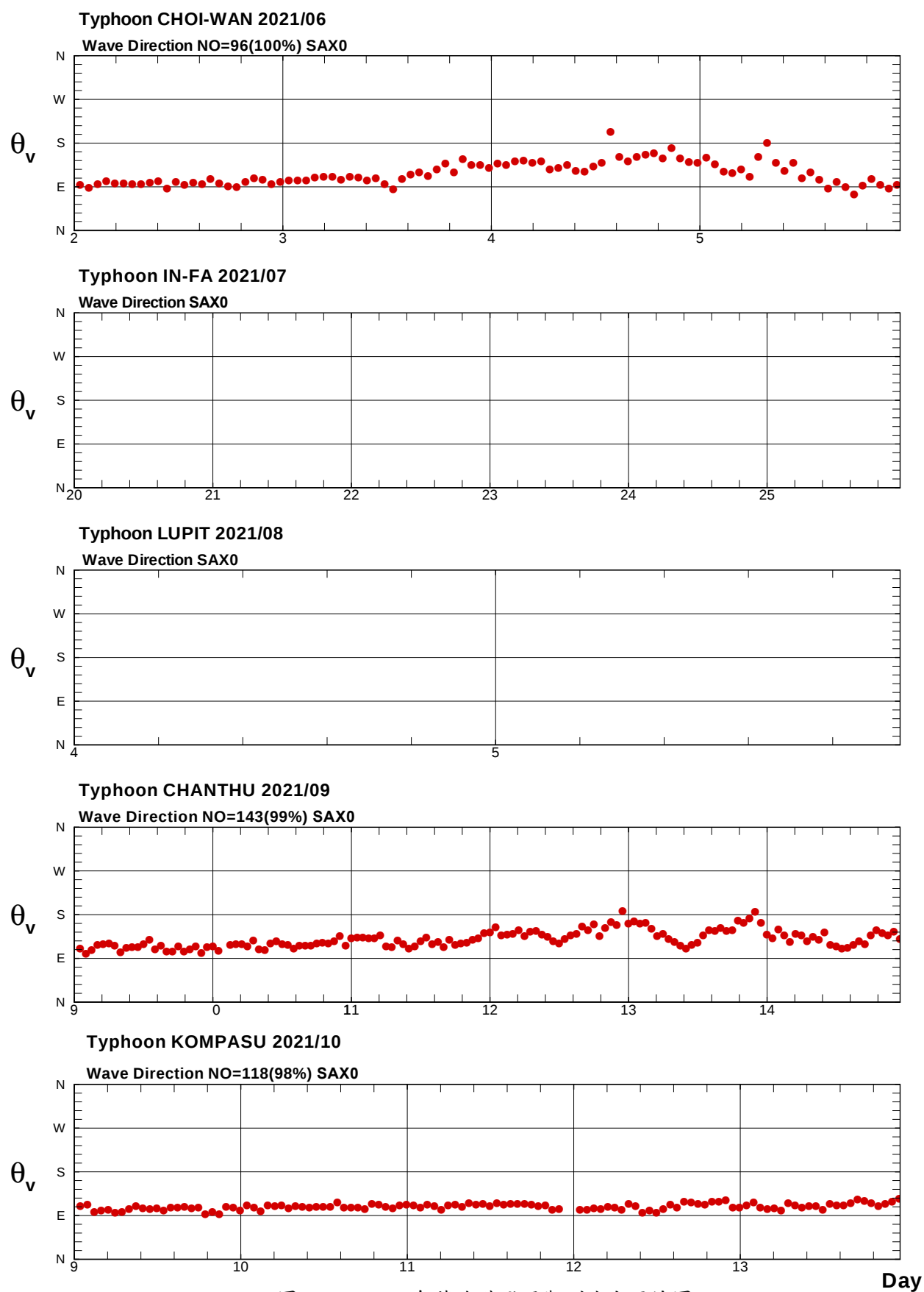
圖4.5b 2021年蘇澳港颱風觀測波向歷線圖
