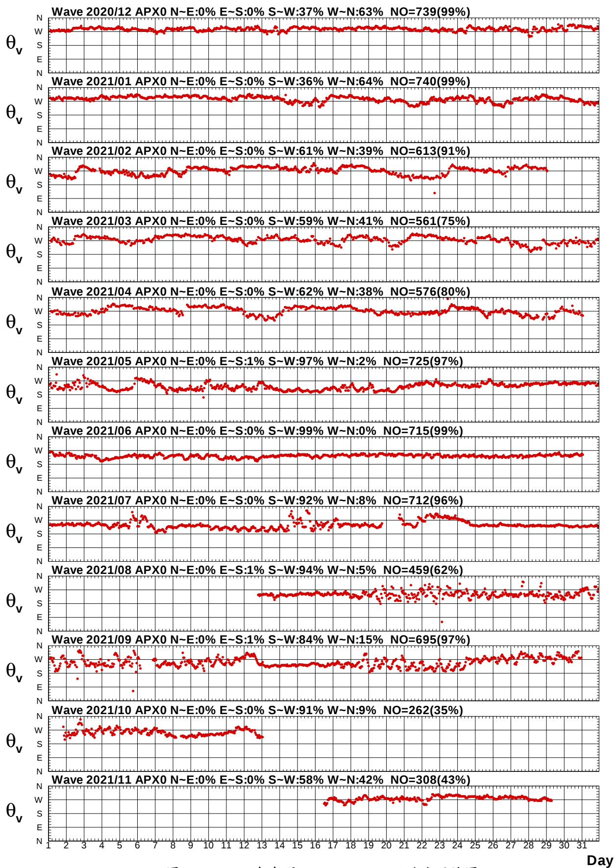
圖7.3c 2021年每月 APAW01H01站波向歷線圖
