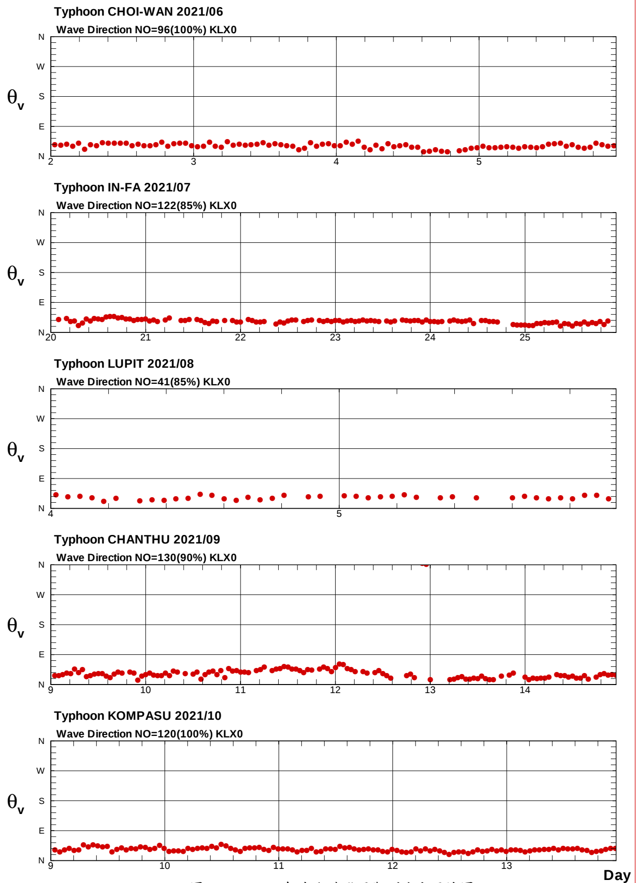
圖3.5b 2021年基隆港颱風觀測波向歷線圖
