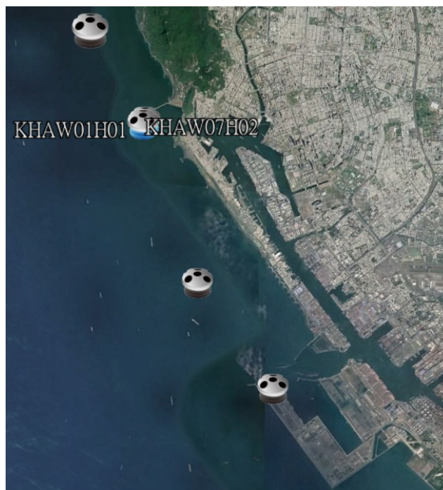
圖 6.1 高雄港波浪測站位置圖
