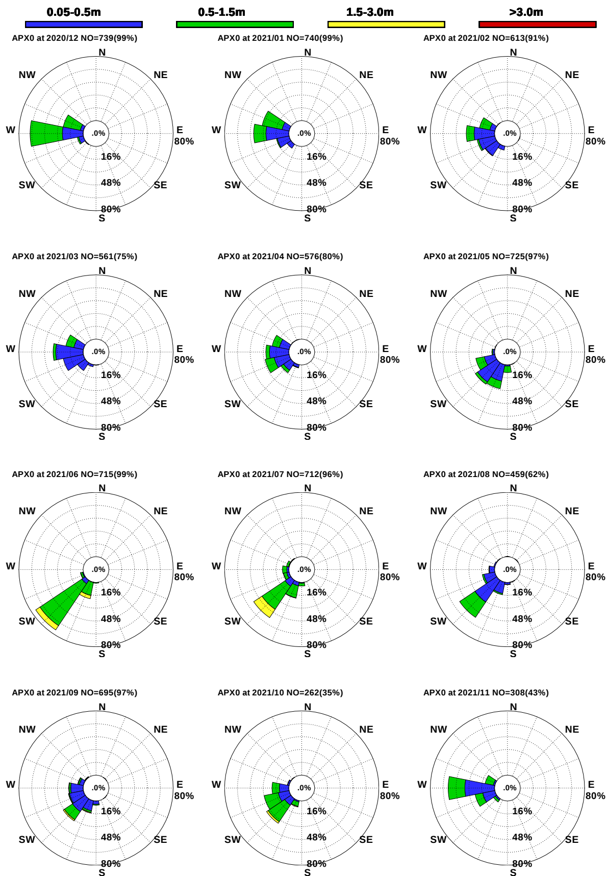
圖7.4a 2021年安平港每月測站 X 觀測浪玫瑰圖
