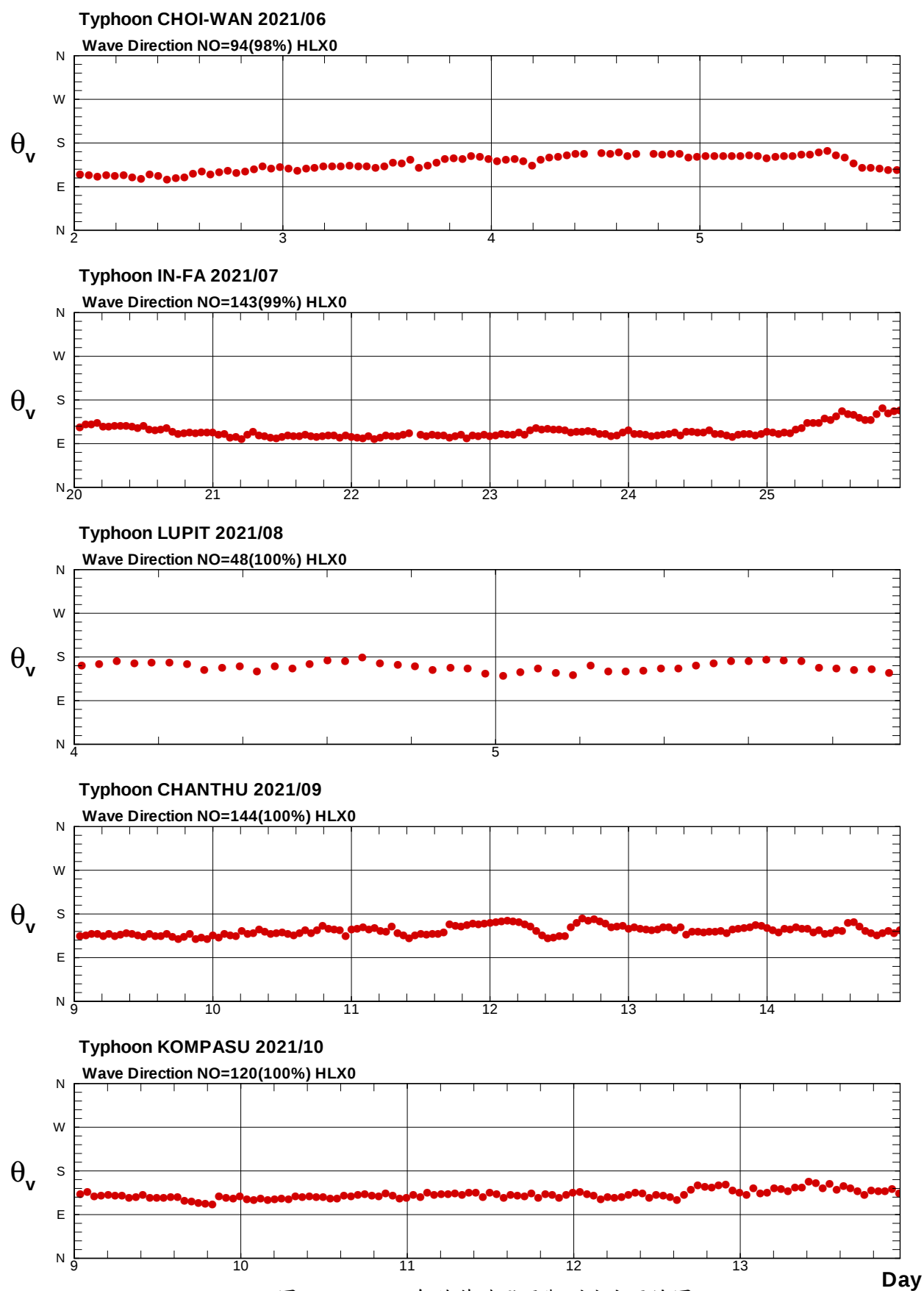
圖5.5b 2021年花蓮港颱風觀測波向歷線圖
