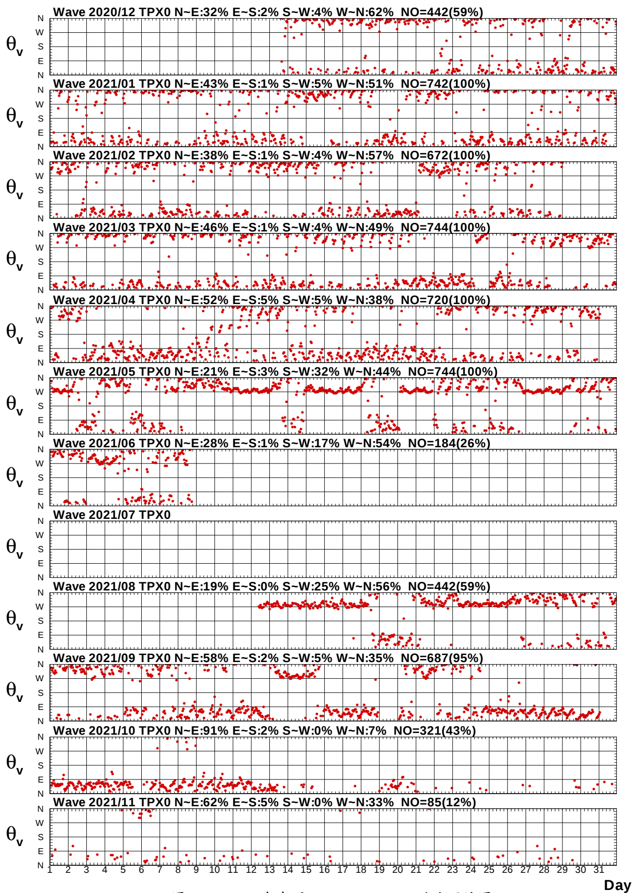
圖2.3c 2021年每月 TPAW01H01 站波向歷線圖
