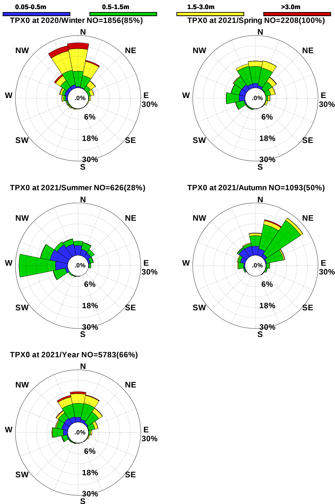
圖2.4b 2021年臺北港每季測站 X 觀測浪玫瑰圖
