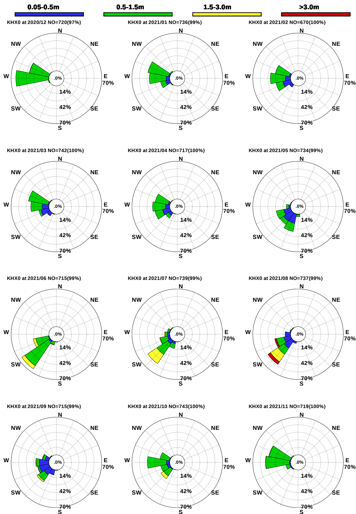
圖6.4a 2021年高雄港每月測站 X 觀測浪玫瑰圖
