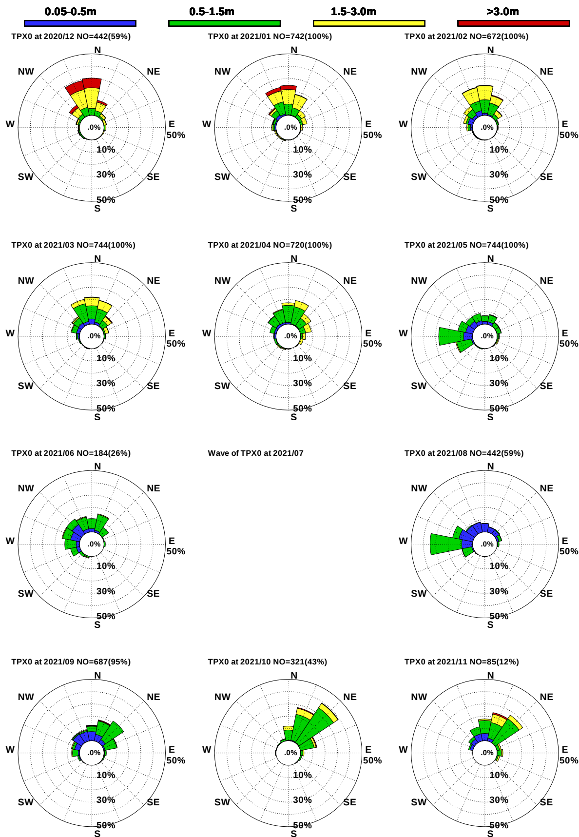
圖2.4a 2021年臺北港每月測站 X 觀測浪玫瑰圖
